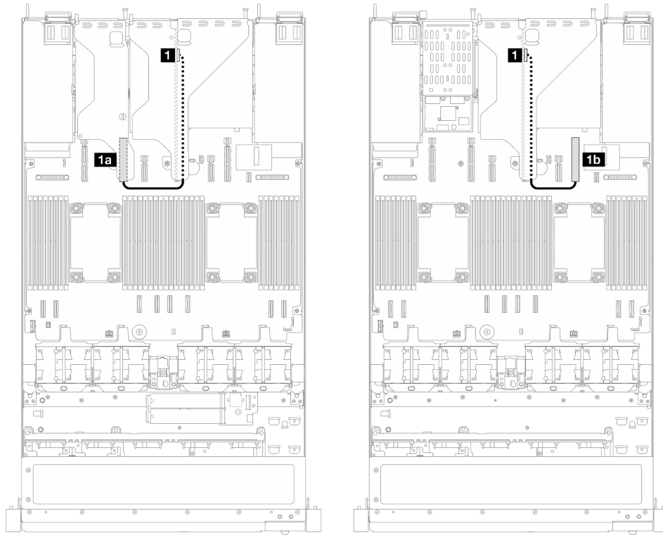
图 12. 背面有线转接卡的线缆布放
