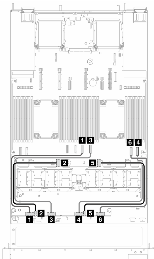
图 23. 配备 8 x 2.5 英寸正面 NVMe 硬盘的板载配置的线缆布放
