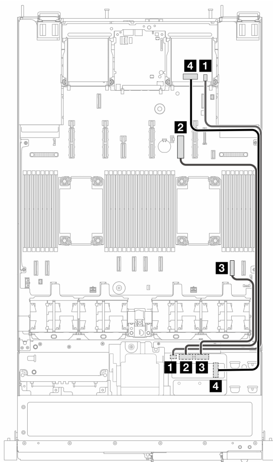
图 8. 配备两个处理器时的 OCP 插转卡线缆布放
