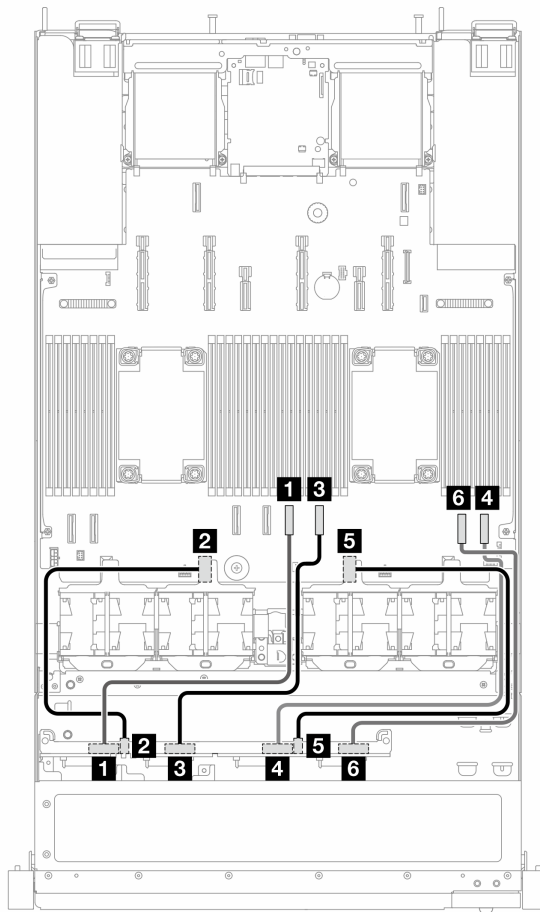
图 21. 配备 8 x 2.5 英寸 NVMe 正面硬盘的板载配置的线缆布放
