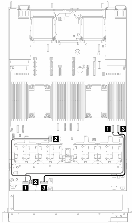
图 18. 配备 4 x 2.5 英寸正面 NVMe 硬盘的板载配置的线缆布放
