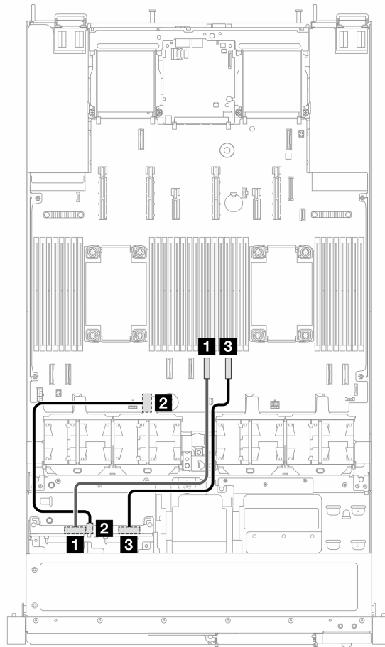
图 15. 配备 4 x 2.5 英寸正面 NVMe 硬盘的板载配置的线缆布放
