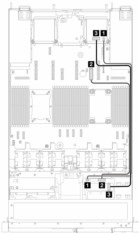
图 7. 配备一个处理器时的 OCP 插转卡线缆布放
