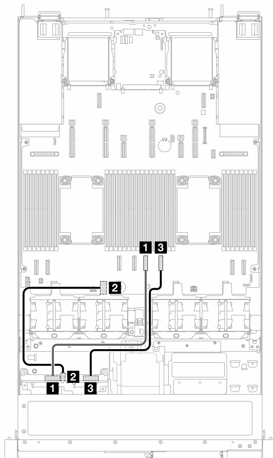
图 16. 配备 4 x 2.5 英寸正面 NVMe 硬盘的板载配置的线缆布放
