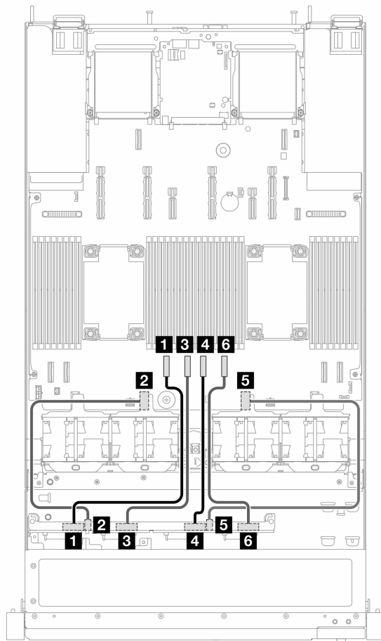
图 20. 配备 8 x 2.5 英寸正面 NVMe 硬盘的板载配置的线缆布放
