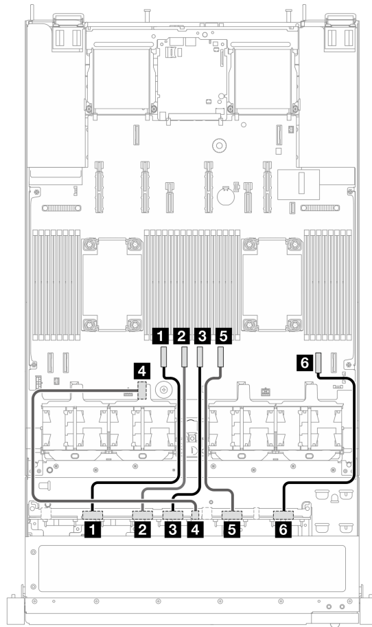
图 24. 配备 10 x 2.5 英寸 NVMe 正面硬盘的板载配置的线缆布放
