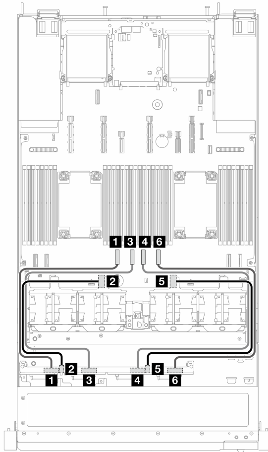
图 22. 配备 8 x 2.5 英寸正面 NVMe 硬盘的板载配置的线缆布放
