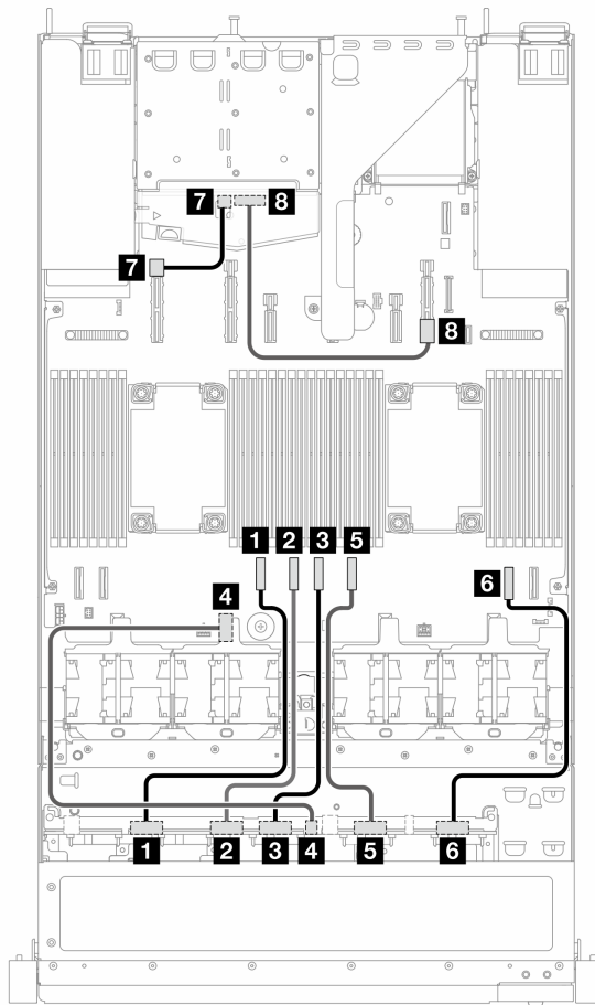
图 26. 配备 12 x 2.5 英寸 NVMe 正面硬盘的板载配置的线缆布放
