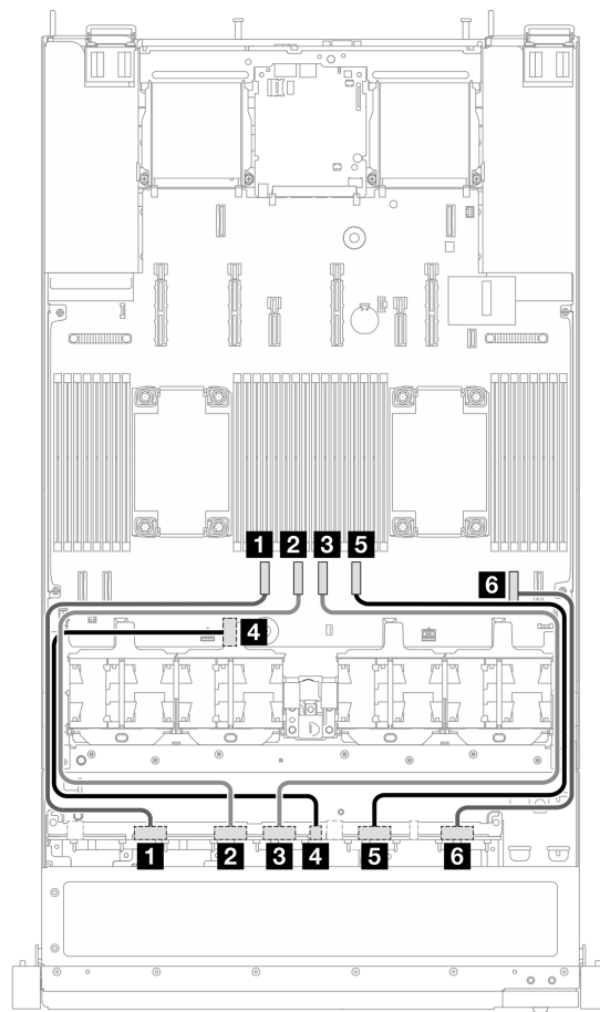
图 25. 液冷 (NeptAir 模块) 的 10 个 NVMe 硬盘的板载布线
