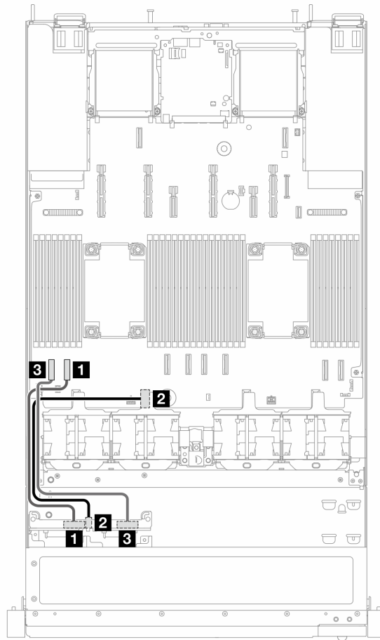
图 19. 配备 4 x 2.5 英寸正面 NVMe 硬盘的板载配置的线缆布放
