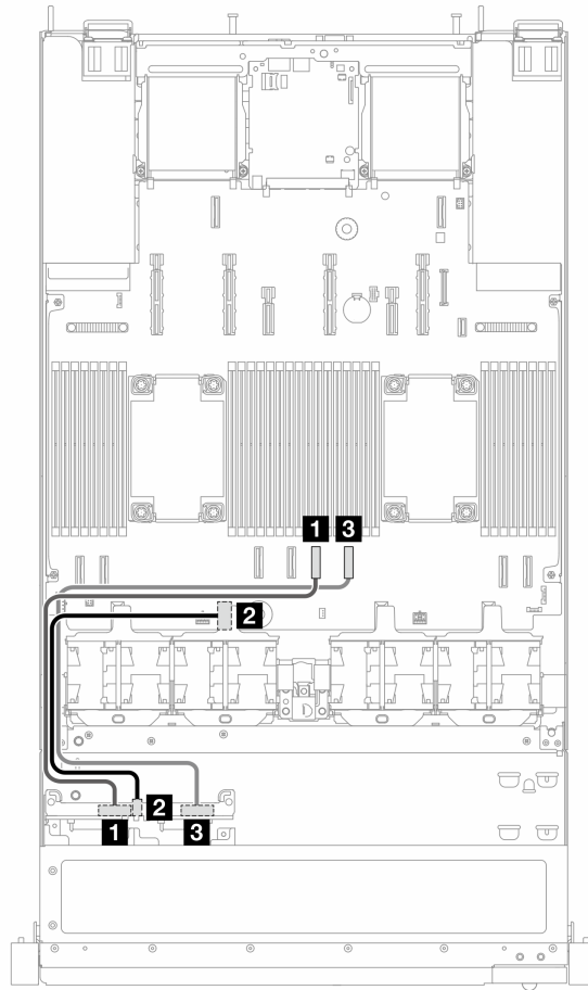
图 17. 液冷 (NeptAir 模块) 配置中的四个 NVMe 硬盘的板载布线
