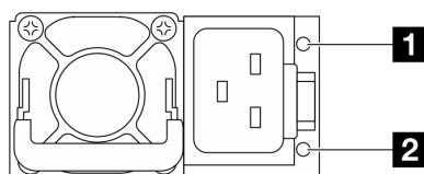
图 20. CRPS Premium 电源模块单元上的 LED
