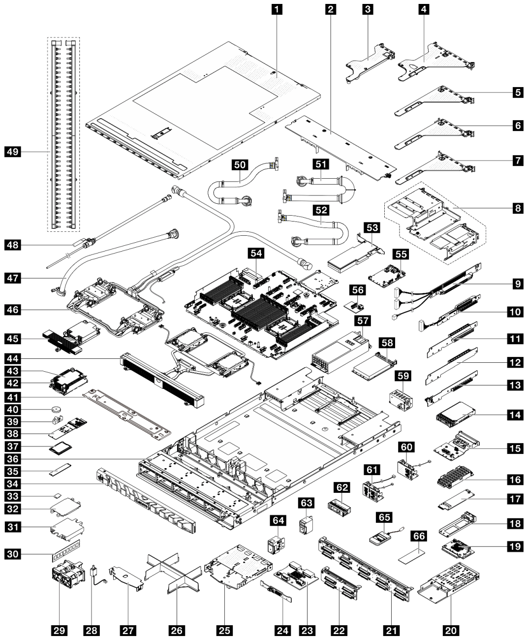
图 28. 服务器组件
