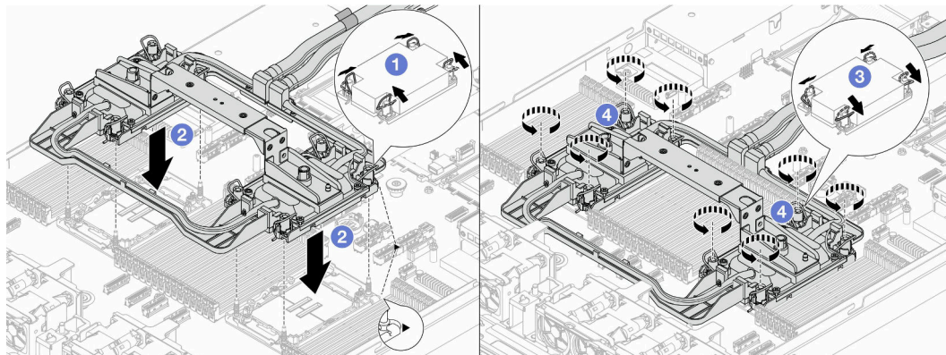
圖例 127. 安裝 NeptCore 模組
