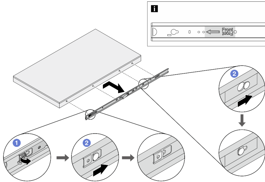
圖例 38. 卸下內滑軌
