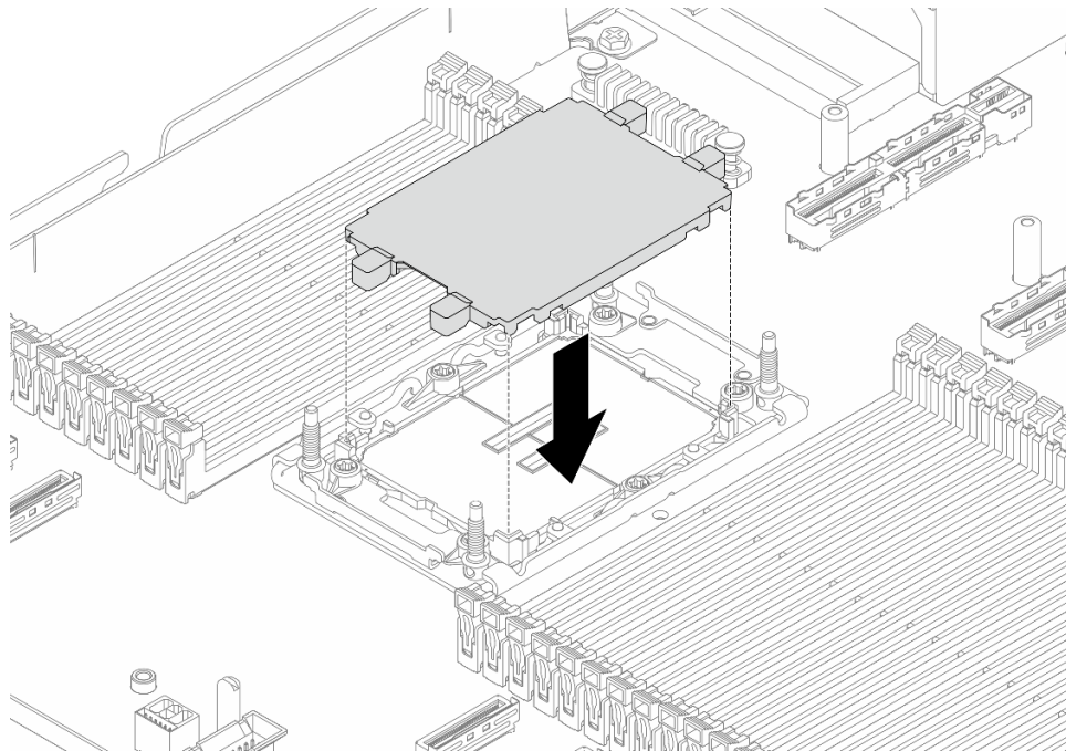
圖例 126. 安裝處理器插座蓋
