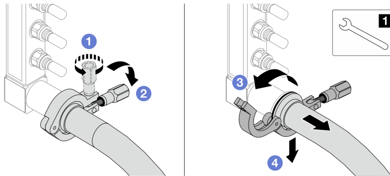
圖例 169. 將歧管與軟管套件分離
