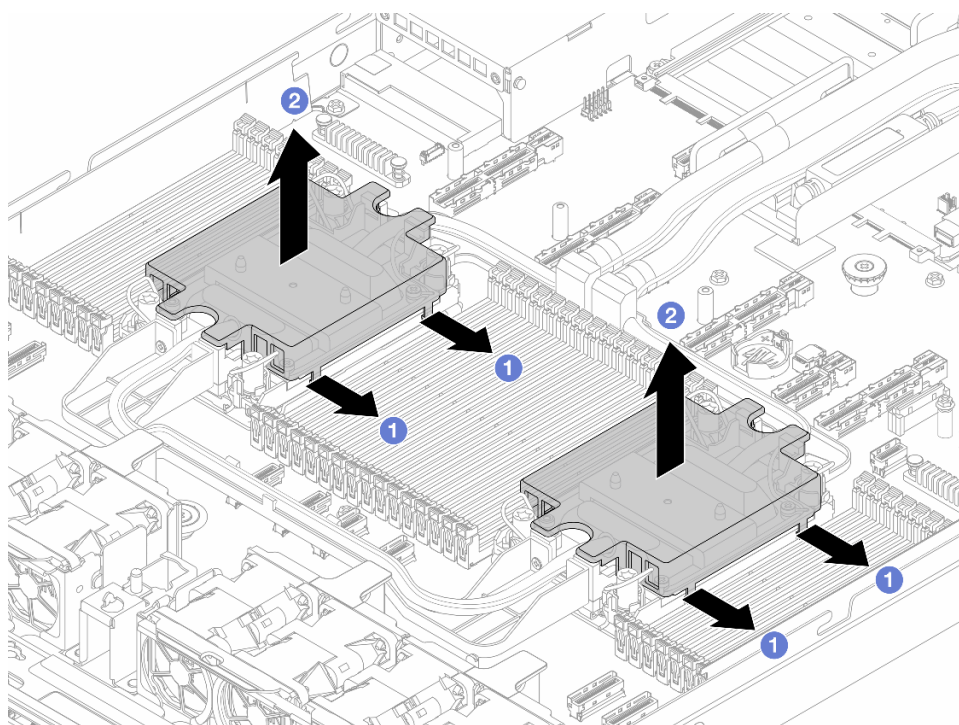
圖例 293. 拆下水冷板蓋
