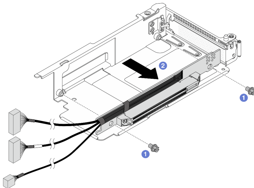
圖例 75. 從半高匣卸下擴充卡
