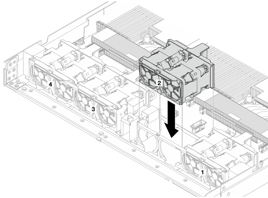
圖例 284. 安裝系統風扇組
