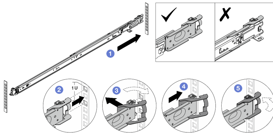
圖例 33. 安裝後方安裝插腳
