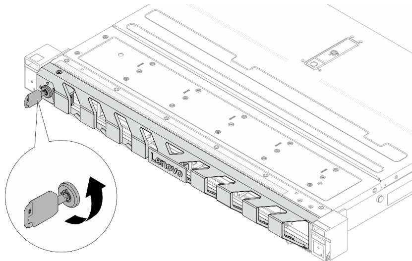
圖例 269. 鎖定安全擋板
