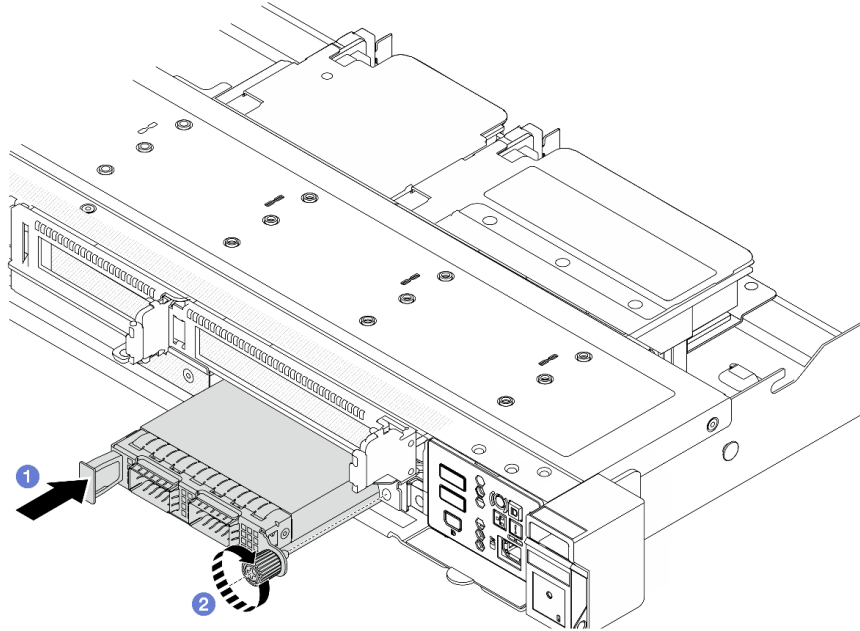
圖例 82. 安裝正面 OCP 模組
