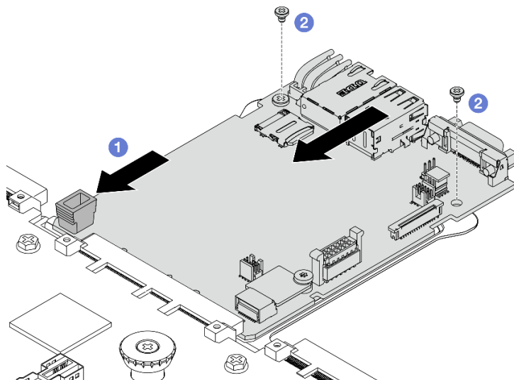
圖例 278. 安裝系統 I/O 板
