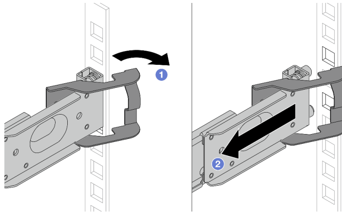
圖例 30. 從後方卸下滑軌
