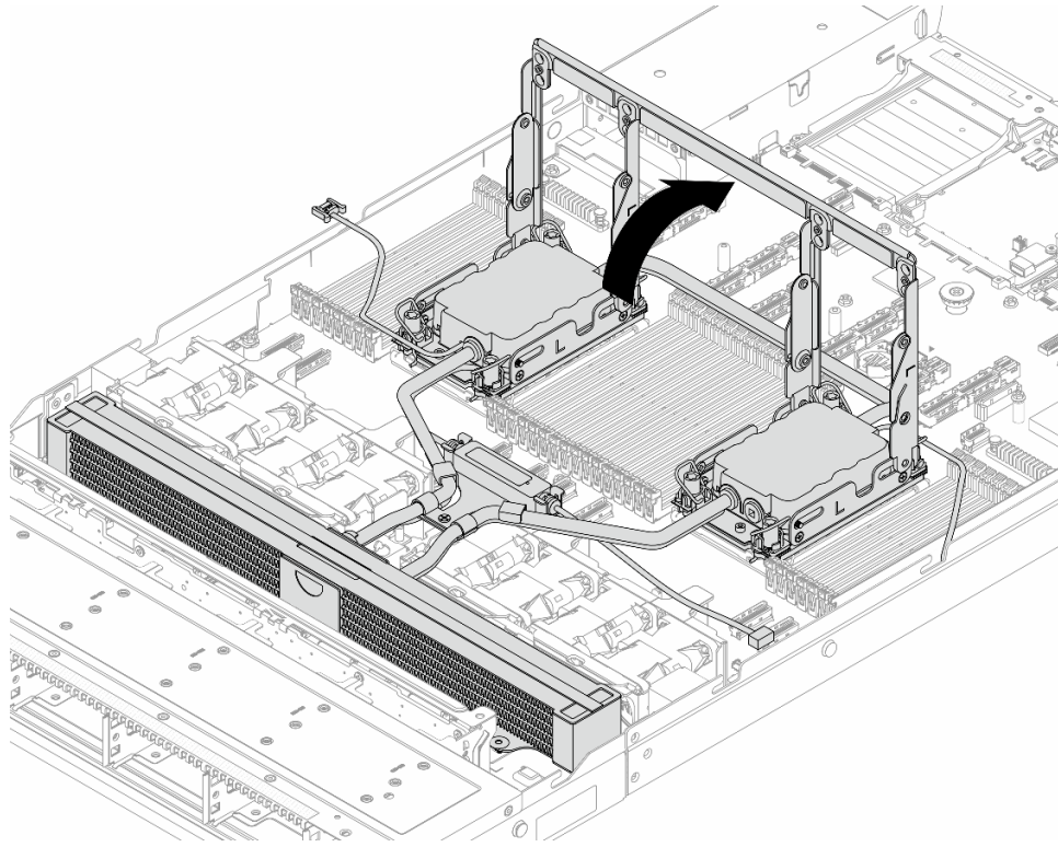
圖例 115. 打開把手
