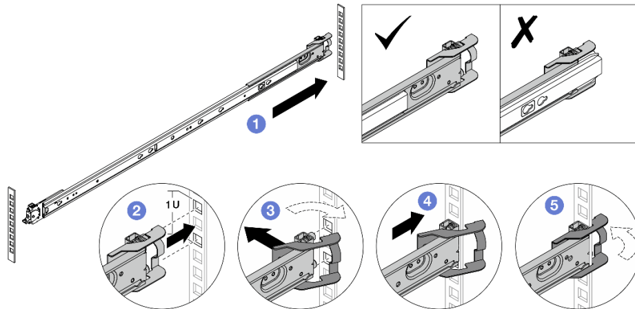
圖例 31. 安裝後方安裝插腳
