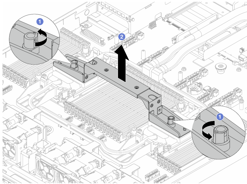
圖例 128. 卸下模組把手
