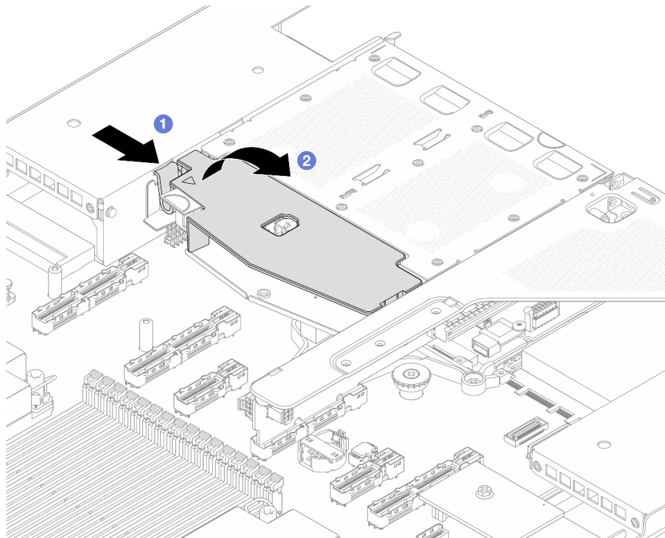
圖例 202. 卸下空氣擋板
