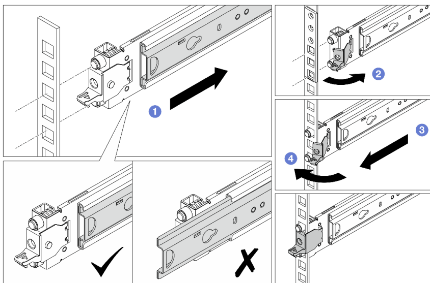
圖例 32. 安裝前方安裝插腳
