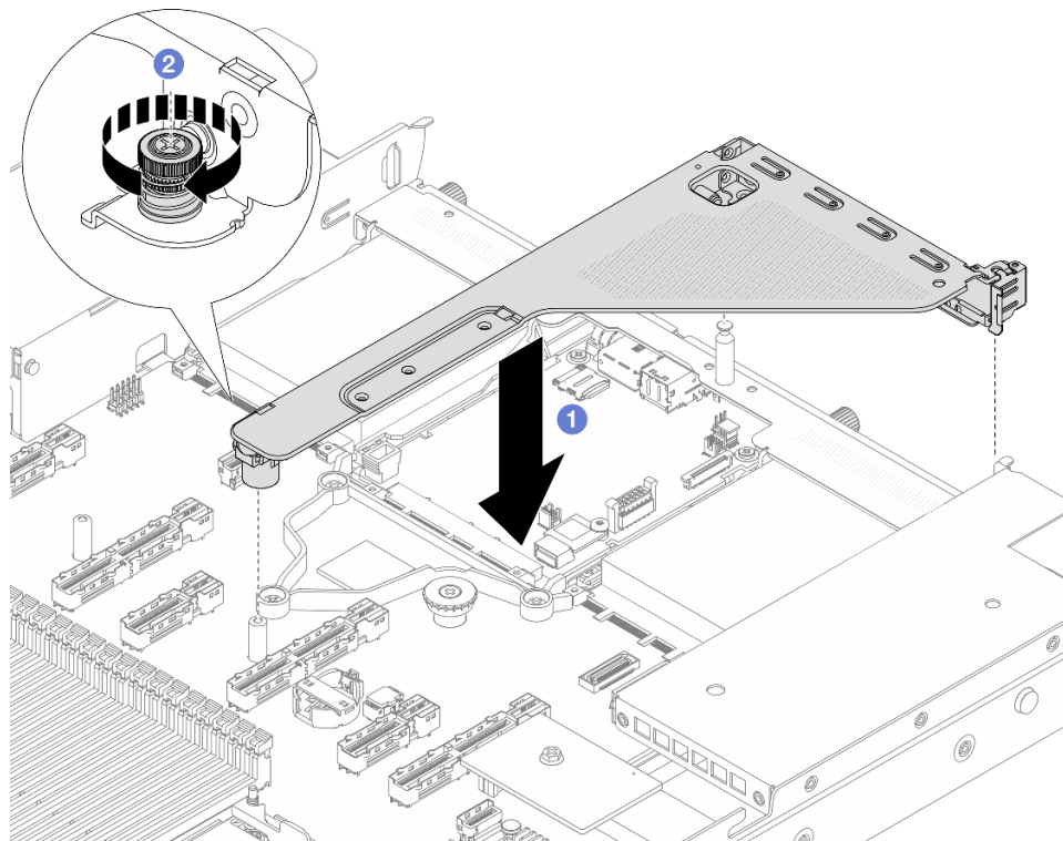
圖例 275. 安裝擴充卡組件
