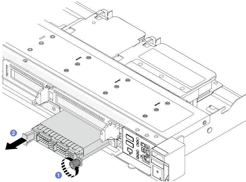
圖例 81. 卸下正面 OCP 模組
