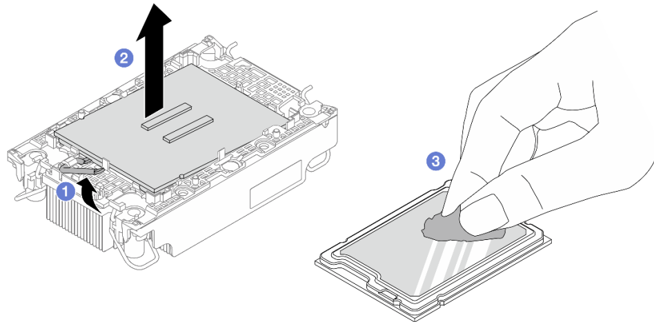
圖例 190. 將處理器與散熱槽和支架分開
