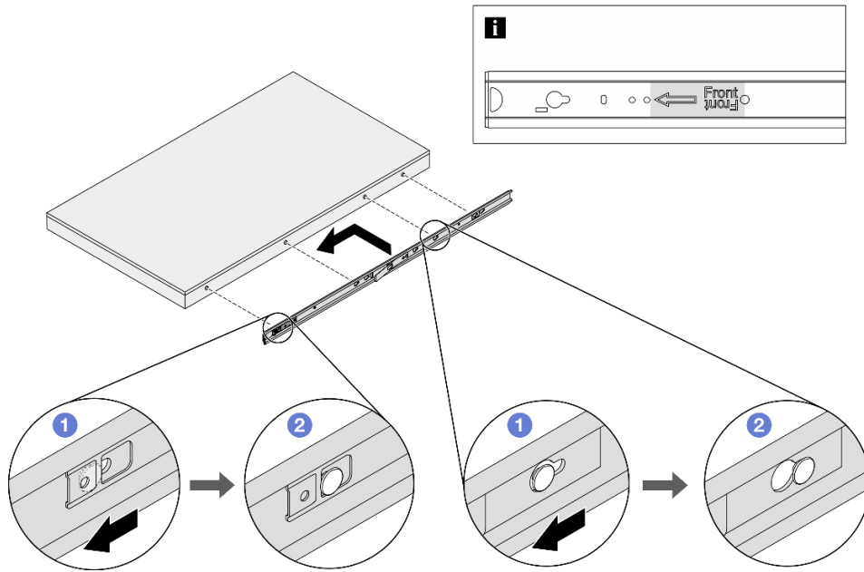
圖例 40. 安裝內滑軌
