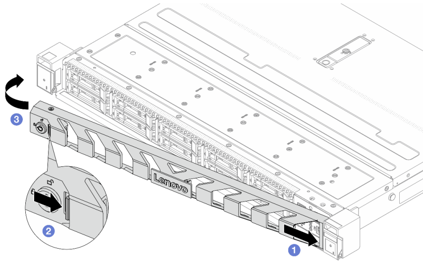
圖例 268. 安裝安全擋板
