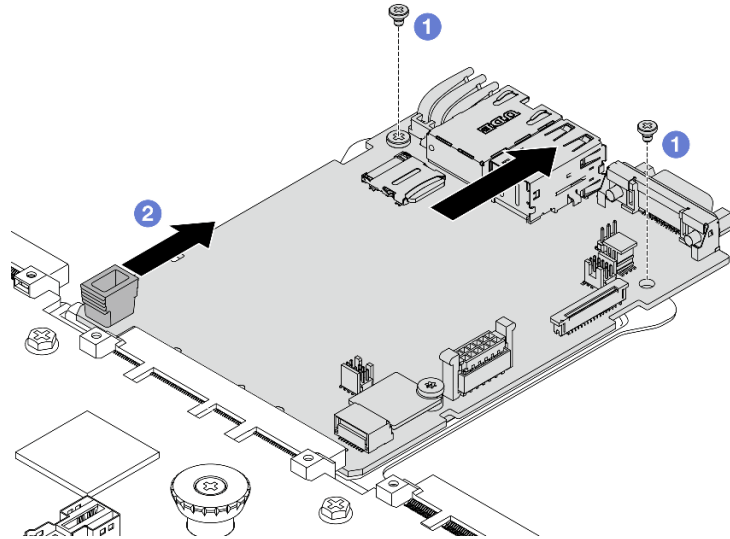
圖例 277. 卸下系統 I/O 板
