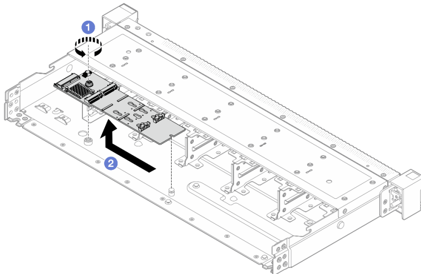
圖例 103. 卸下 M.2 模組
