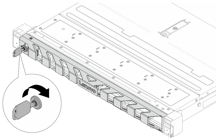
圖例 265. 解鎖安全擋板
