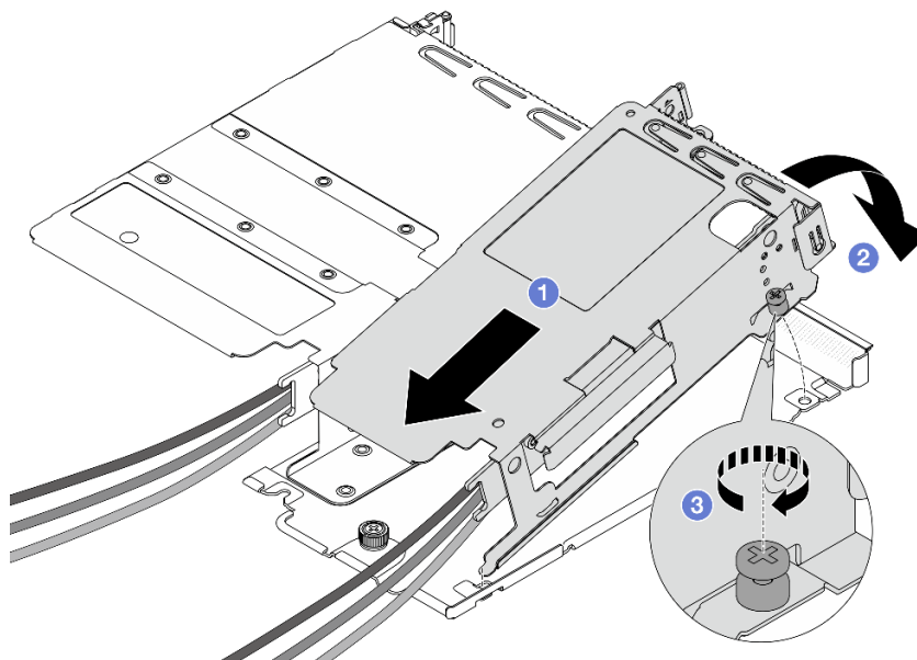
圖例 80. 組裝兩個擴充卡匣
