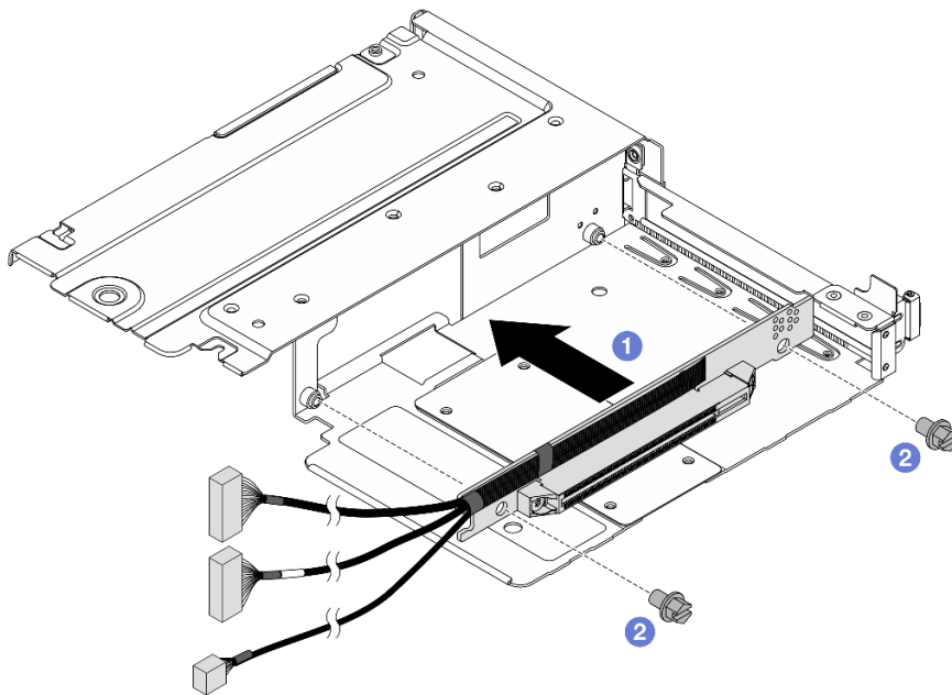
圖例 78. 將擴充卡安裝到全高匣
