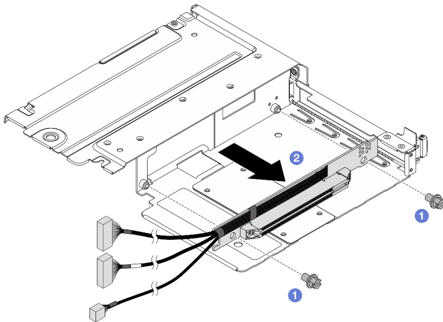
圖例 76. 從全高匣卸下擴充卡
