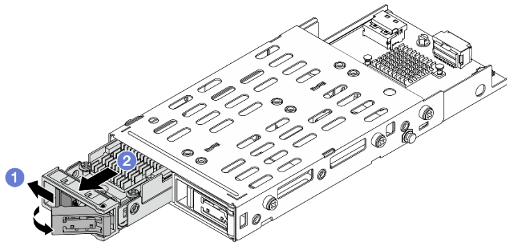
圖例 214. 卸下背面 M.2 硬碟組件
