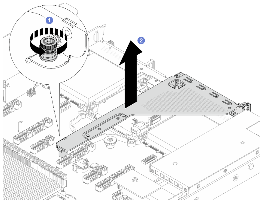
圖例 270. 卸下擴充卡托架
