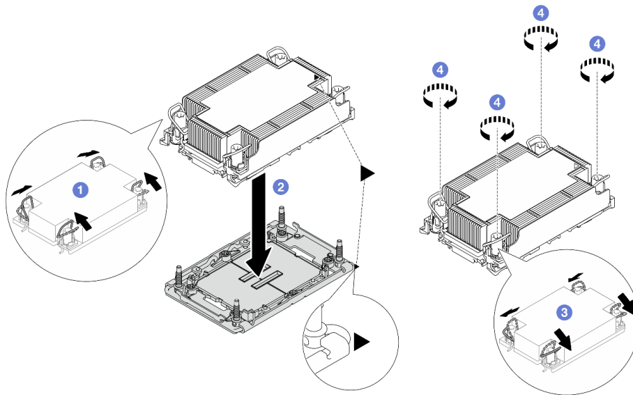
圖例 197. 安裝 PHM
