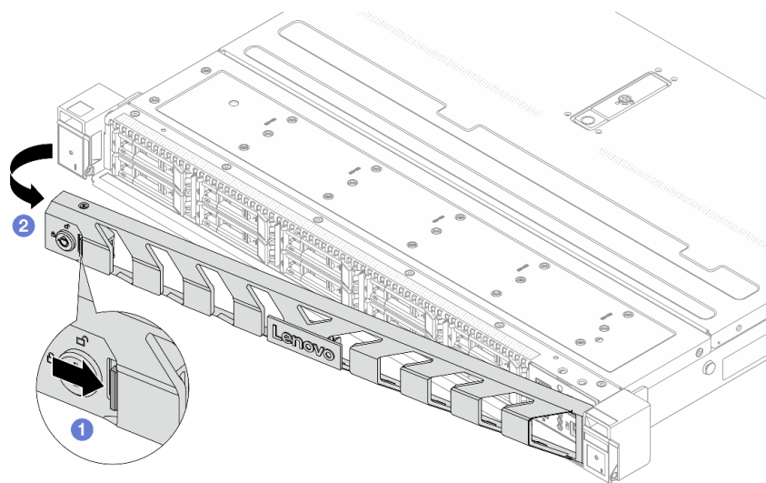
圖例 266. 卸下安全擋板
