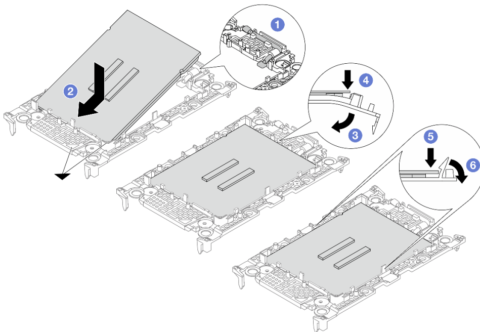
圖例 193. 安裝處理器支架
