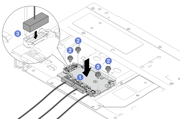
圖例 84. 安裝正面 OCP 轉插卡
