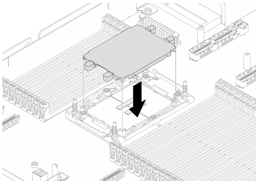
圖例 117. 安裝處理器插座蓋
