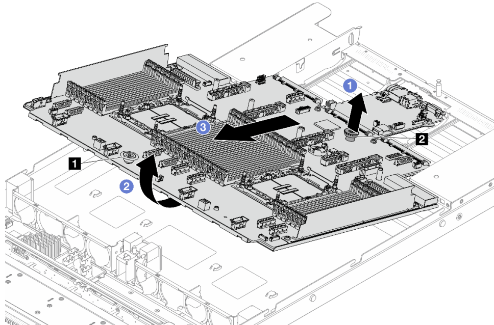
圖例 279. 卸下主機板組件
