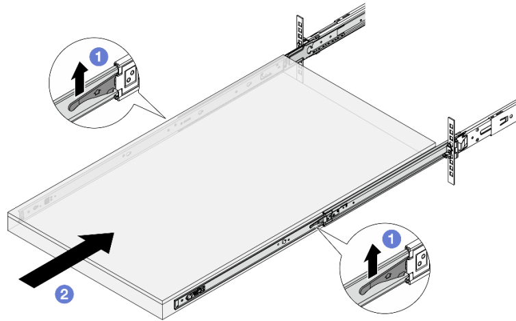
圖例 53. 鎖定滑軌，並將伺服器滑入
