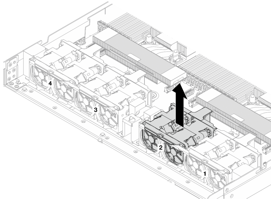
圖例 283. 卸下系統風扇組
