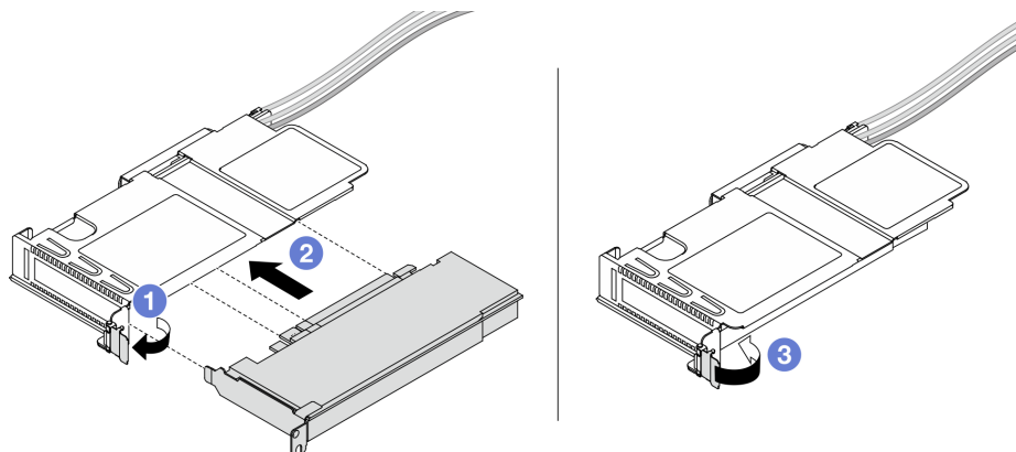
圖例 79. 安裝 PCIe 配接卡
