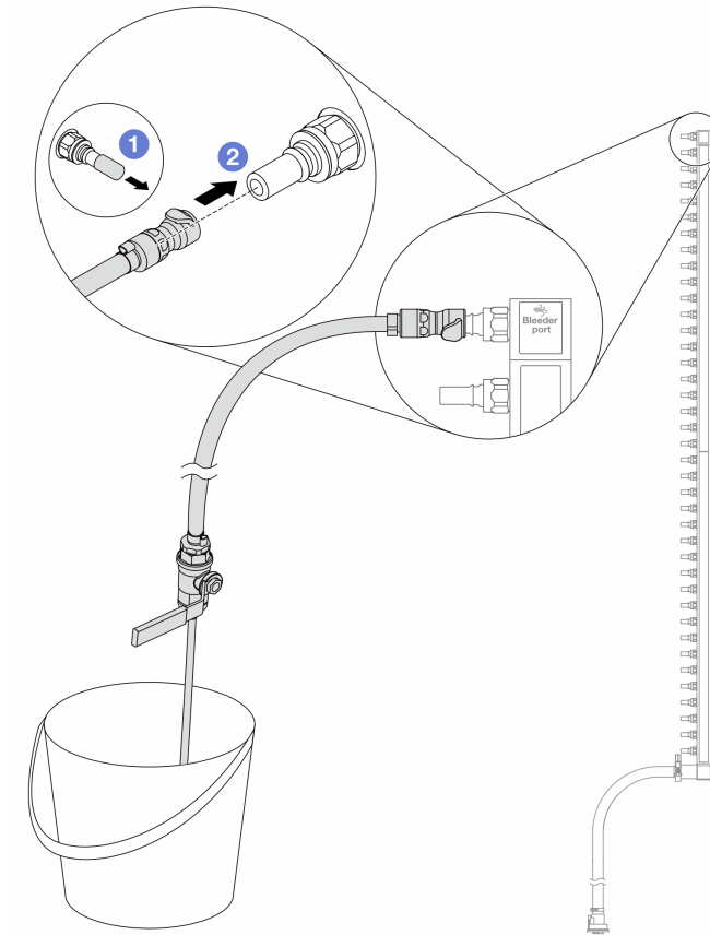
圖例 167. 在回流側安裝洩放套件
