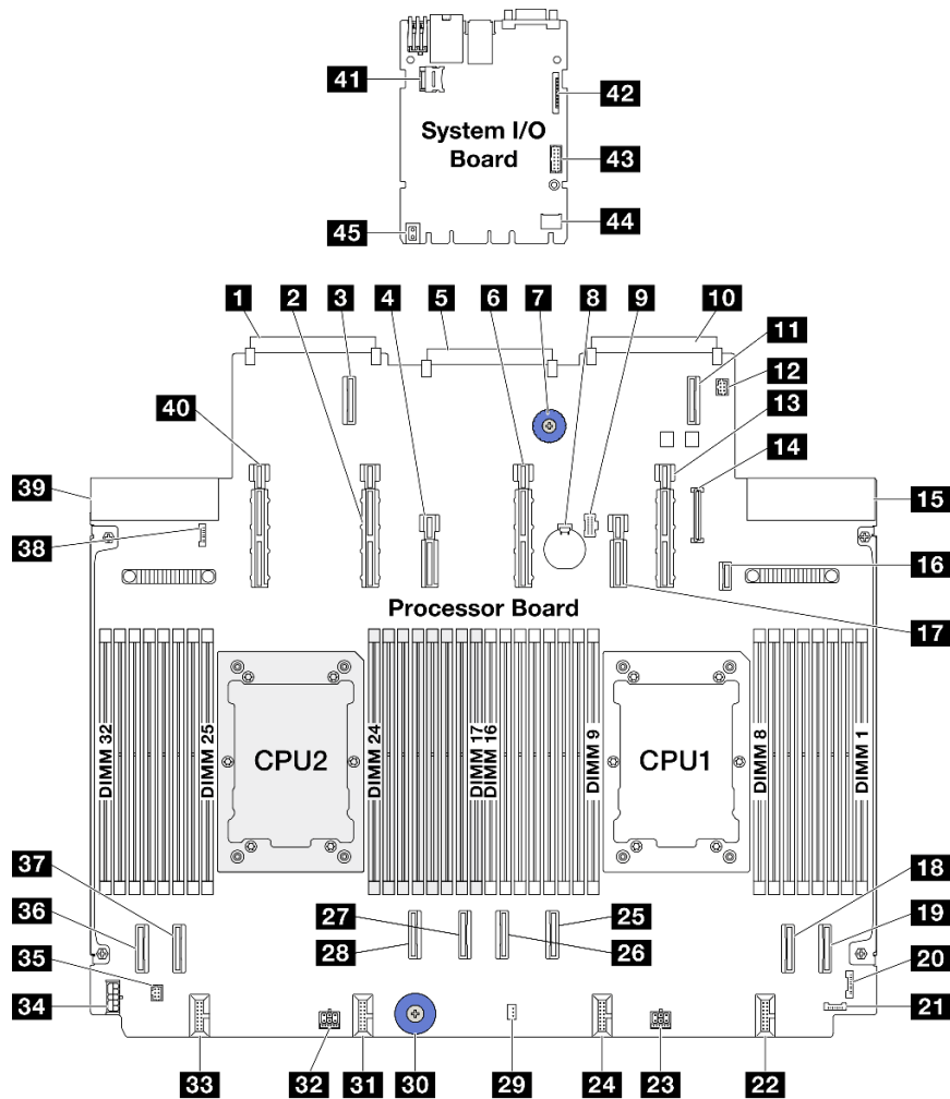
圖例 291. 主機板組件接頭
