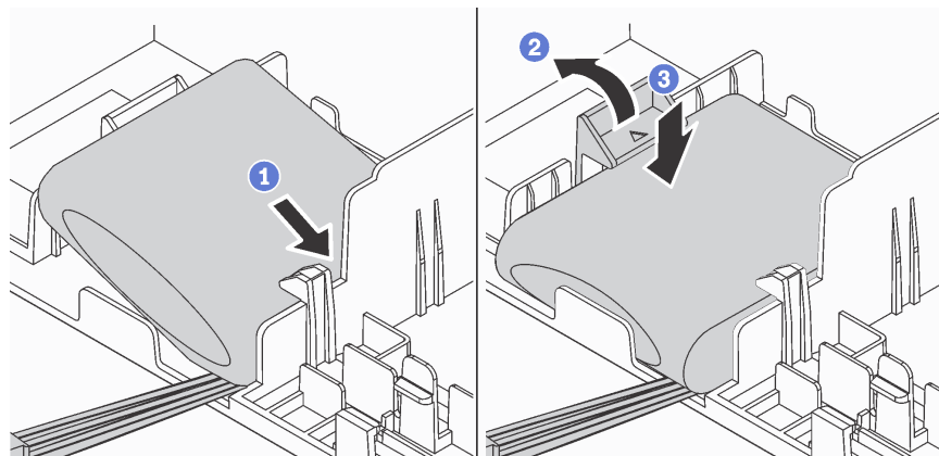
Figura 82. Instalación de un módulo supercondensador RAID en la parte inferior del deflector de aire
