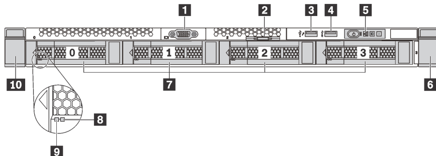
Figura 7. Vista frontal de modelos de servidor con cuatro bahías de unidad de 3,5 pulgadas
