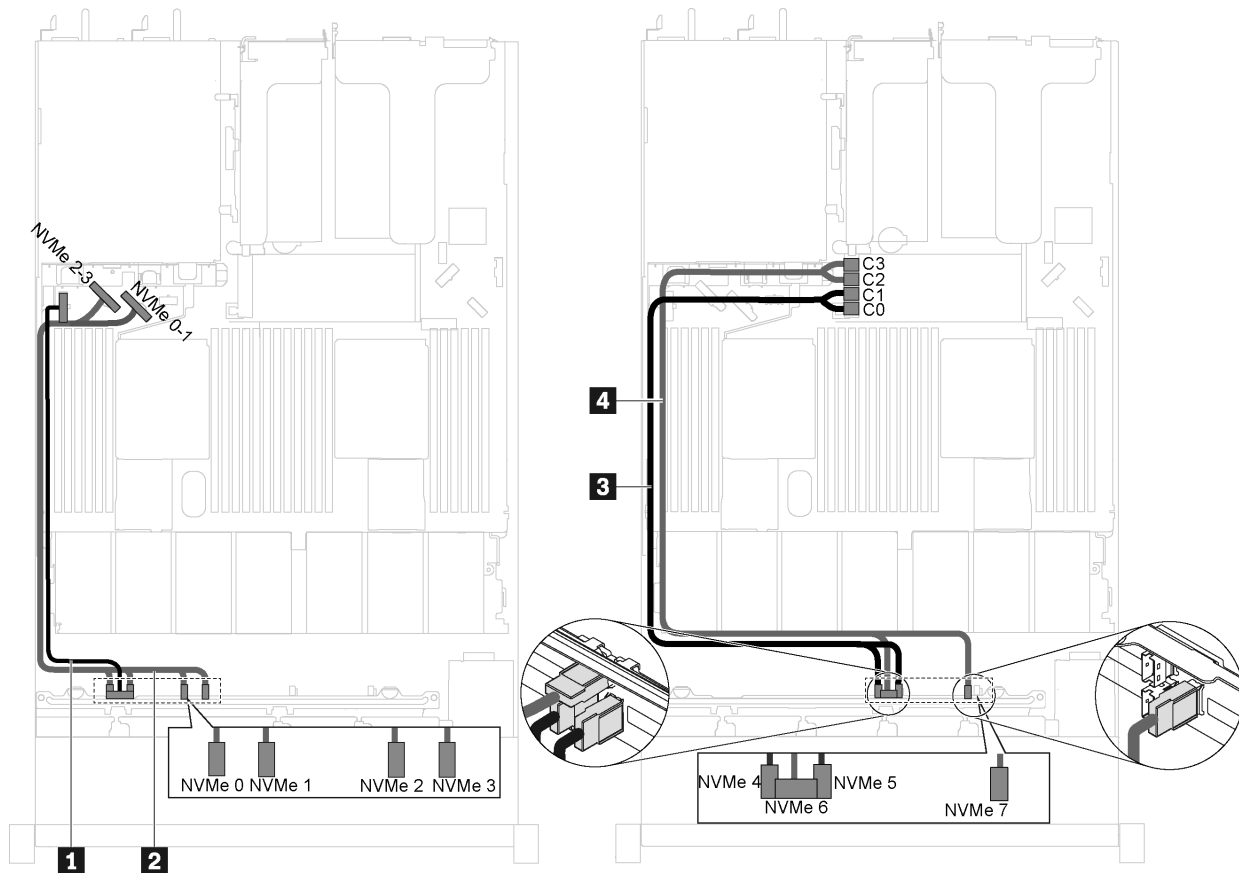
Figura 42. Disposición de cables para modelos de servidor con ocho unidades NVMe de 2,5 pulgadas y un adaptador de conmutador NVMe de 810-4P en la ranura del adaptador RAID
