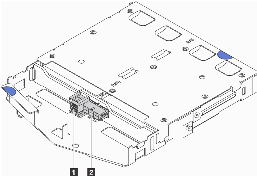
Figura 60. Conectores de la placa posterior
