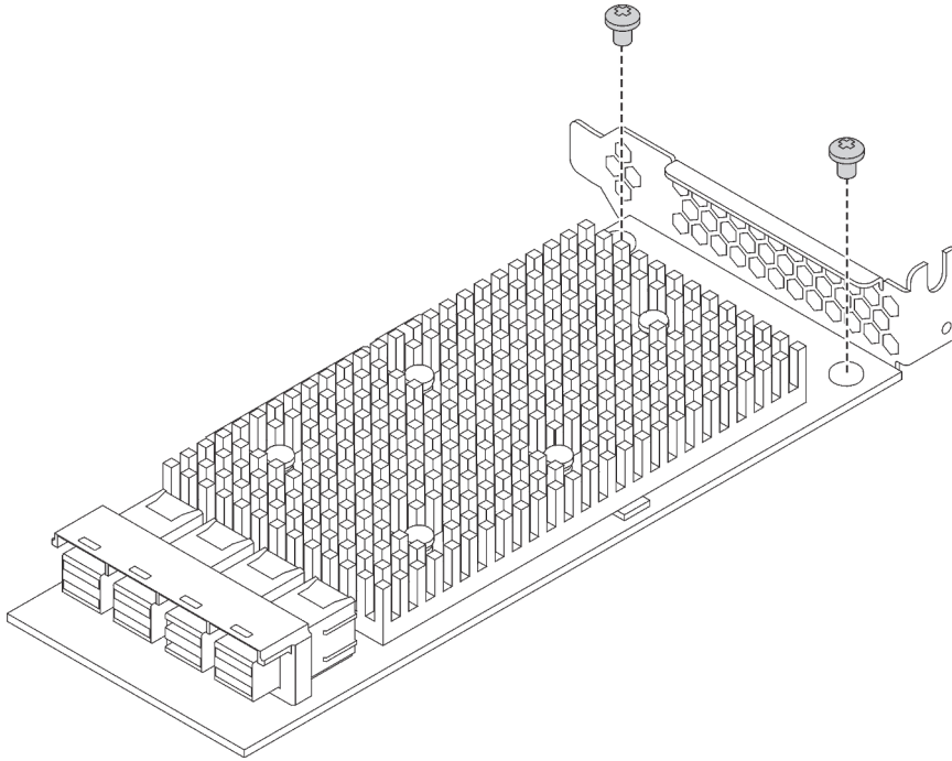
Figura 77. Instalación de la abrazadera de bajo perfil al adaptador RAID
