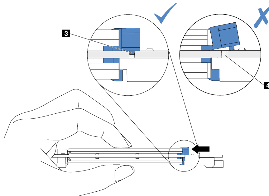
Figura 65. Instrucciones para deslizar el elemento de sujeción
