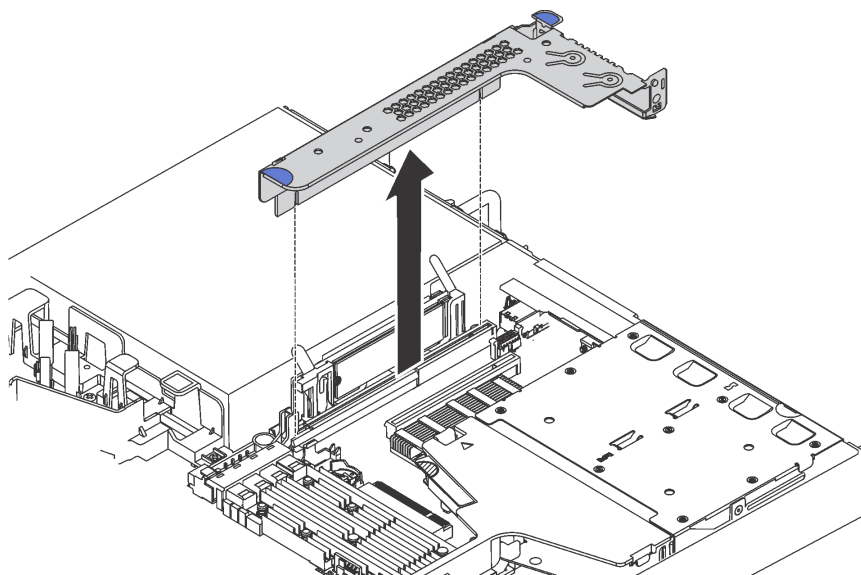
Figura 78. Extracción del conjunto de expansión
