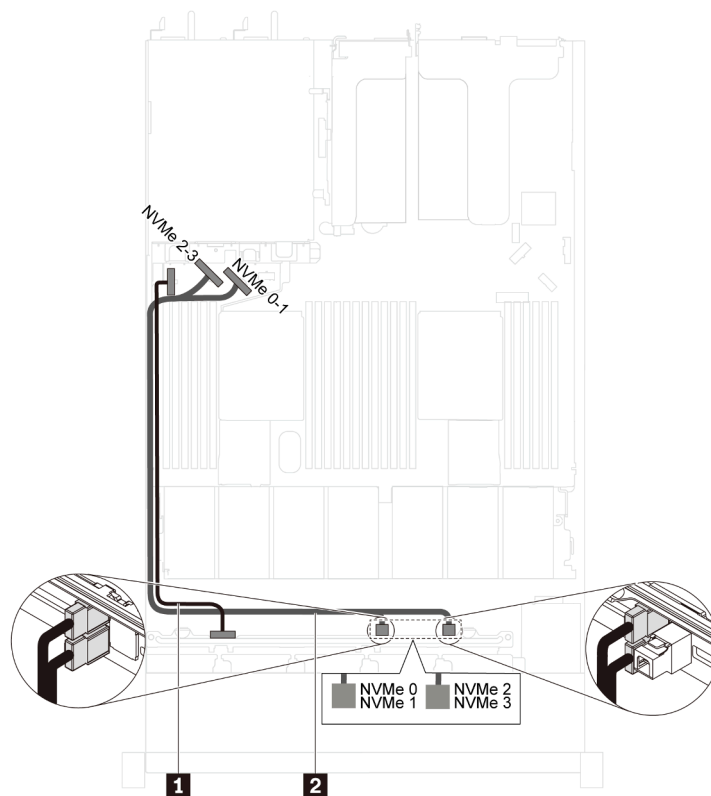
Figura 37. Disposición de los cables para los modelos de servidor con cuatro unidades NVMe de 2,5 pulgadas y sin adaptador RAID
