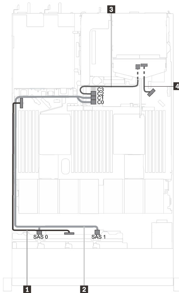
Figura 28. Disposición de los cables para los modelos de servidor con ocho unidades SAS/SATA de 2,5 pulgadas, un adaptador HBA/RAID 16i y el conjunto de unidad posterior
