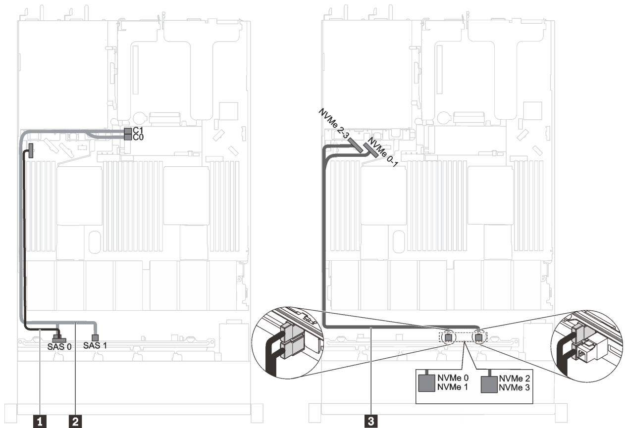
Figura 32. Disposición de los cables de modelos de servidor con seis unidades SAS/SATA de 2,5 pulgadas, cuatro unidades NVMe de 2,5 pulgadas y un adaptador HBA/RAID 8i
