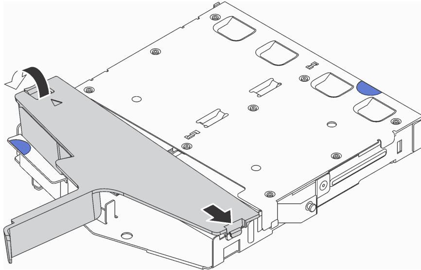
Figura 61. Instalación del deflector de aire
