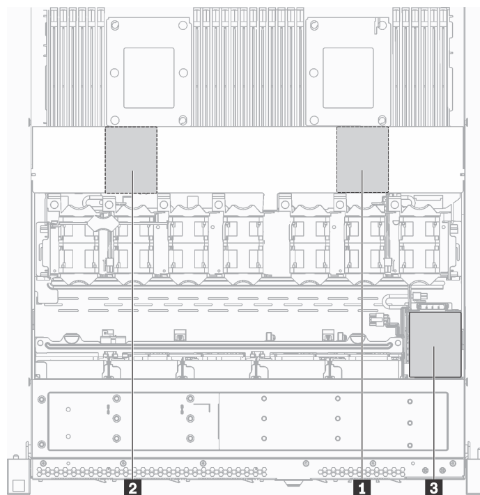
Figura 83. Ubicación del módulo supercondensador RAID
