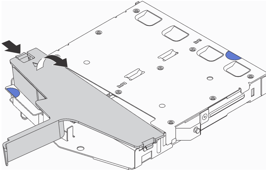
Figura 59. Extracción del deflector de aire
