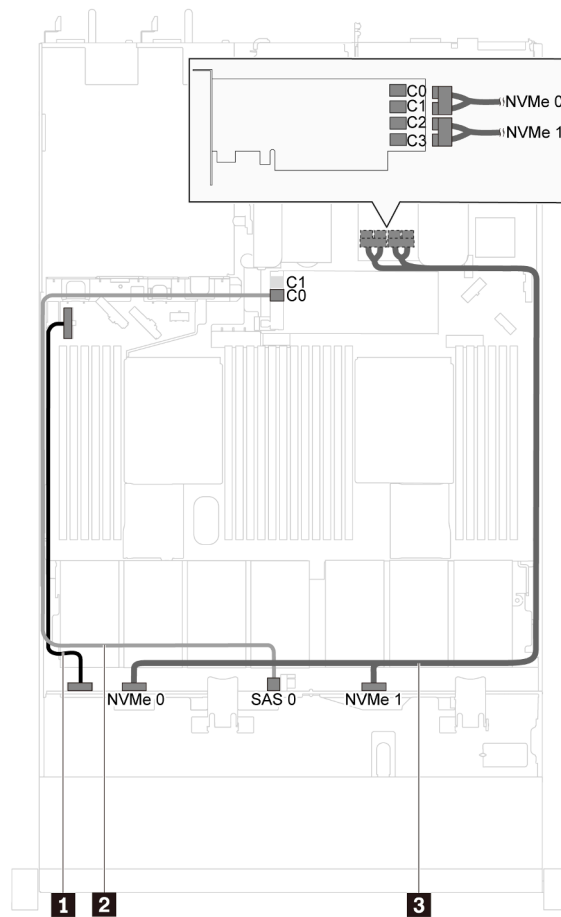
Figura 25. Disposición de cables para modelos de servidor con cuatro unidades SAS/SATA/NVMe de 3,5 pulgadas y un adaptador de conmutador NVMe de 1610-4P en PCIe ranura 2
