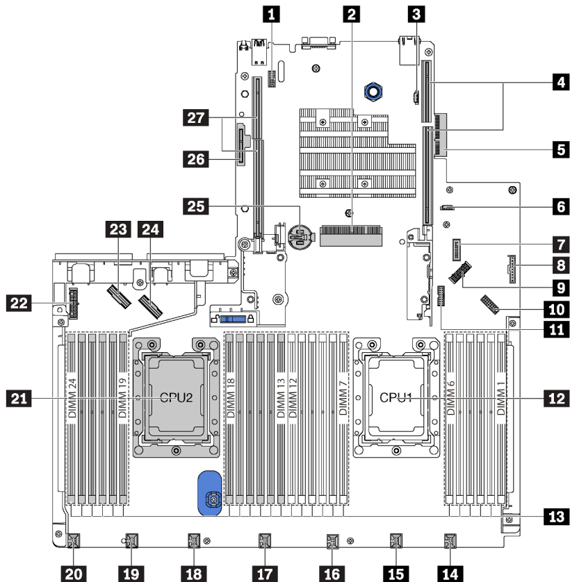
Figura 18. Componentes de la placa del sistema
