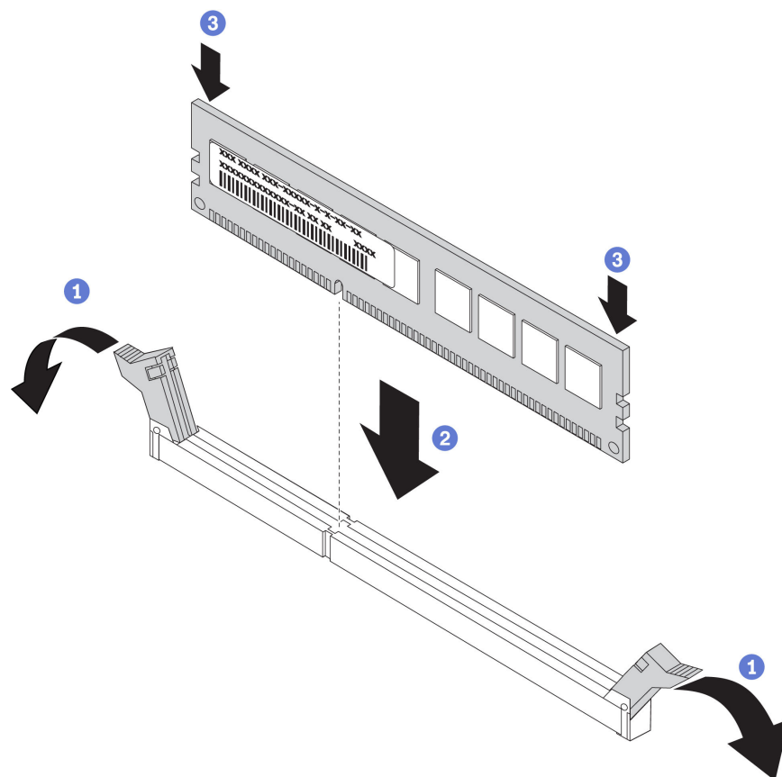
Figura 52. Instalación de un módulo de memoria
