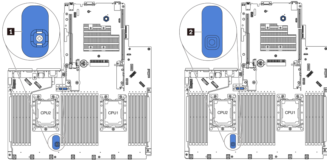
Figura 4. Dos tipos de placa del sistema
