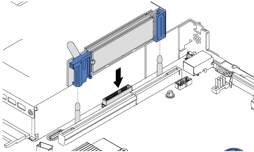
Figura 66. Instalación de la placa posterior M.2
