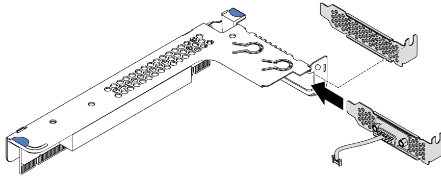
Figura 79. Instalación de módulo de puerto serie
