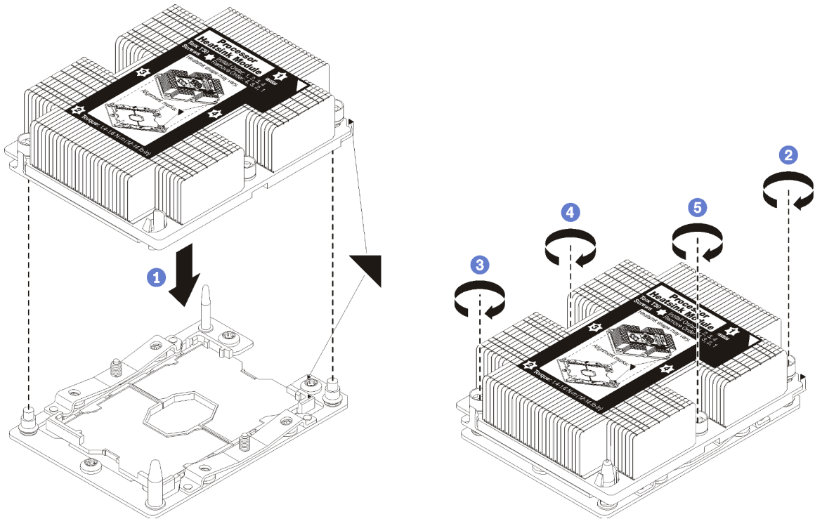
Figura 50. Instalación de un PHM
