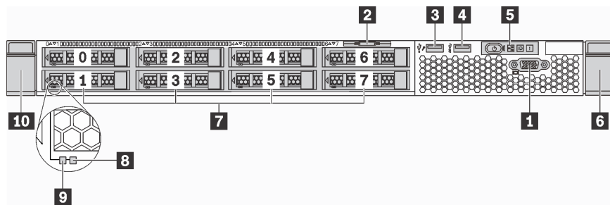
Figura 8. Vista frontal de modelos de servidor con ocho bahías de unidad de 2,5 pulgadas
