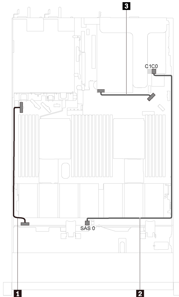
Figura 21. Distribución de cables para modelos de servidor con cuatro unidades SAS/SATA de 3,5 pulgadas y una GPU de altura completa y longitud media
