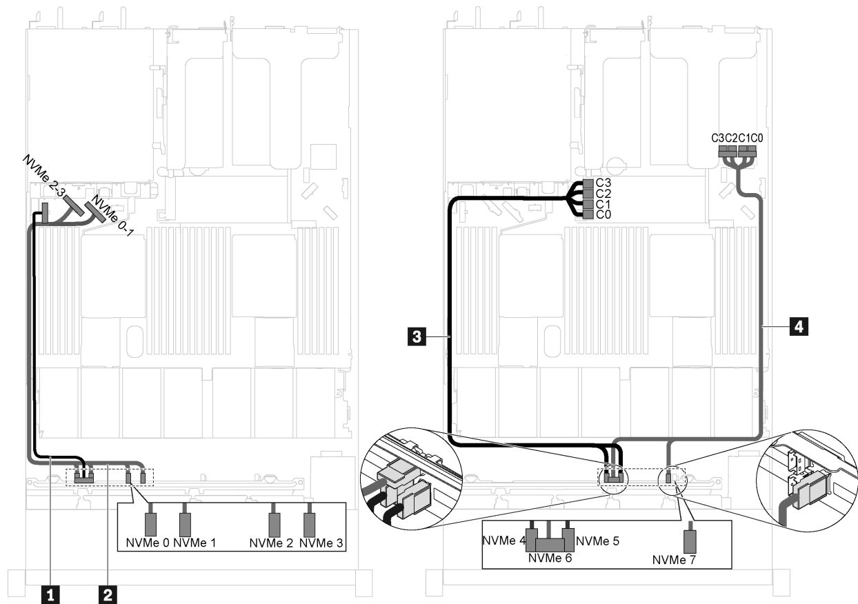
Figura 43. Disposición de cables para modelos de servidor con ocho unidades NVMe de 2,5 pulgadas, un adaptador de conmutador NVMe 810-4P en la ranura de PCIe 1 y un adaptador de conmutador NVMe 810-4P en la ranura de adaptador RAID
