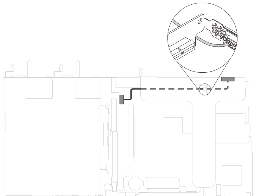
Figura 80. Disposición de los cables para el módulo de puerto serie instalado en la ranura de PCIe 1
