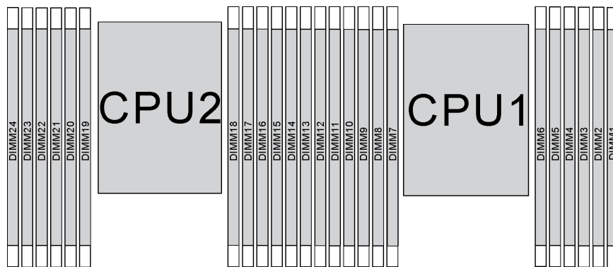
Figura 53. ranuras de módulos de memoria en la placa del sistema
