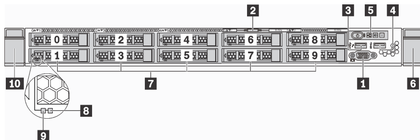
Figura 9. Vista frontal de modelos de servidor con diez bahías de unidad de 2,5 pulgadas
