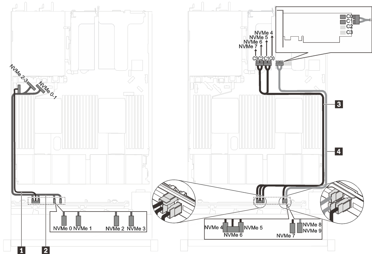
Figura 39. Disposición de cables para modelos de servidor con diez unidades NVMe de 2,5 pulgadas, un adaptador de conmutador NVMe 1610-4P en la ranura de PCIe 2 y un adaptador de conmutador NVMe 1610-4P en la ranura de PCIe 3
