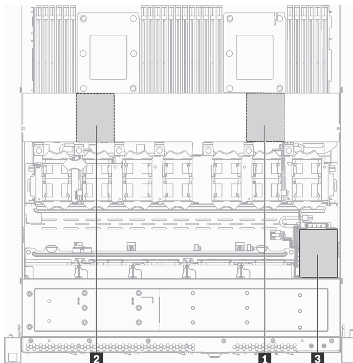
Figura 81. Ubicación del módulo supercondensador RAID
