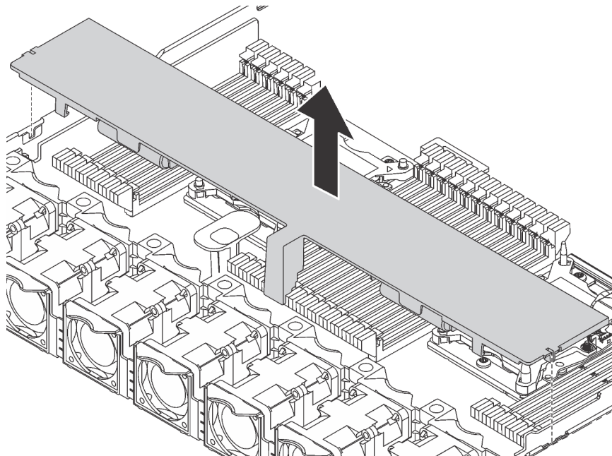
Figura 49. Extracción del deflector de aire
