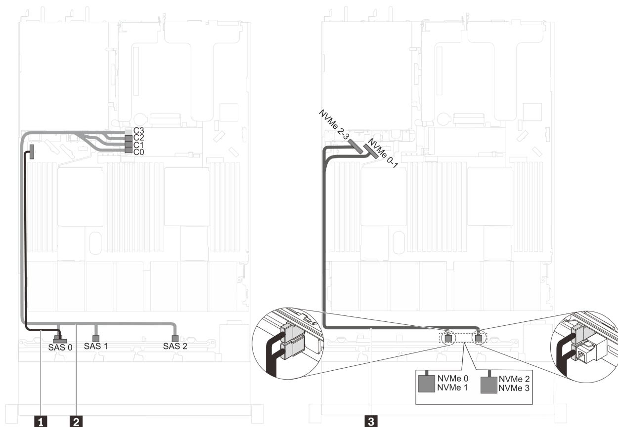
Figura 35. Disposición de los cables de modelos de servidor con procesadores Intel Xeon 6154, 6254 y 6240Y cuatro unidades SAS/SATA/NVMe de 2,5 pulgadas y un adaptador HBA/RAID 16i
