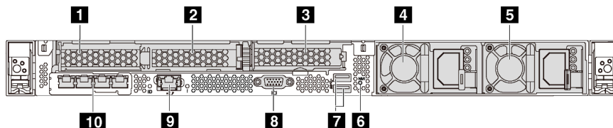
Figura 11. Vista posterior de modelos de servidor con tres ranuras de PCIe
