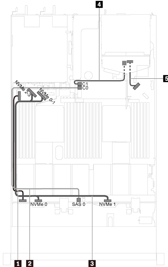
Figura 23. Modelos de servidor con cuatro unidades SAS/SATA/NVMe de 3,5 pulgadas y conjunto de unidad posterior
