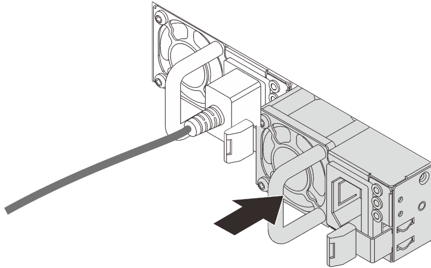
Figura 57. Instalación de una fuente de alimentación de intercambio en caliente
