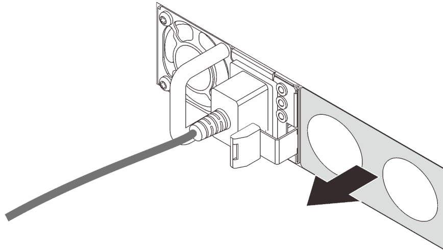
Figura 56. Extracción de relleno de fuente de alimentación de intercambio en caliente
