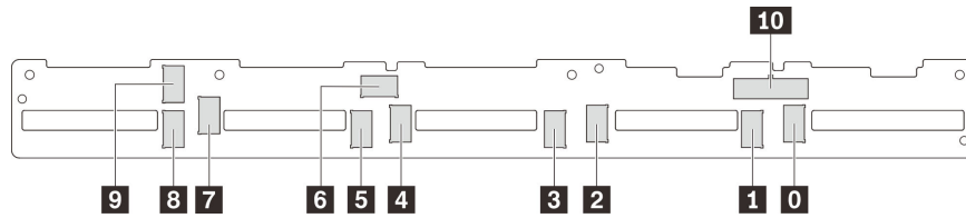
Figura 38. Conectores de la placa posterior para diez unidades NVMe de 2,5 pulgadas
