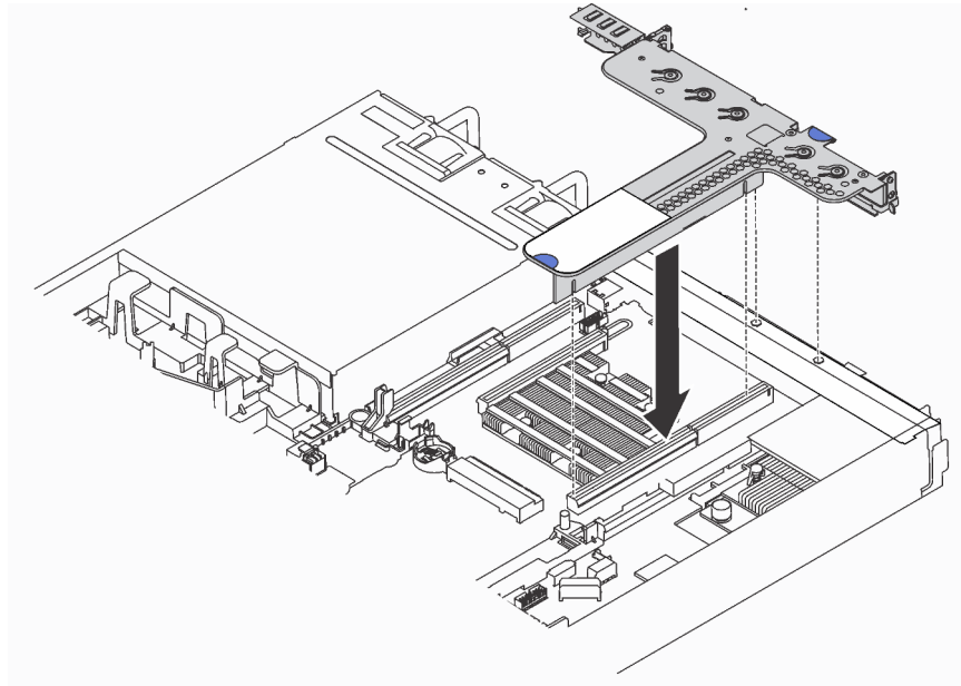
Figura 75. Instalación del conjunto de expansión
