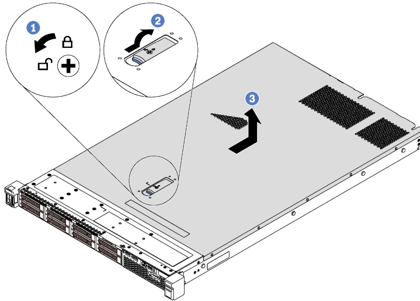
Figura 48. Extracción de la cubierta superior
