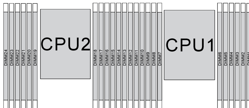
Figura 54. ranuras de módulos de memoria en la placa del sistema
