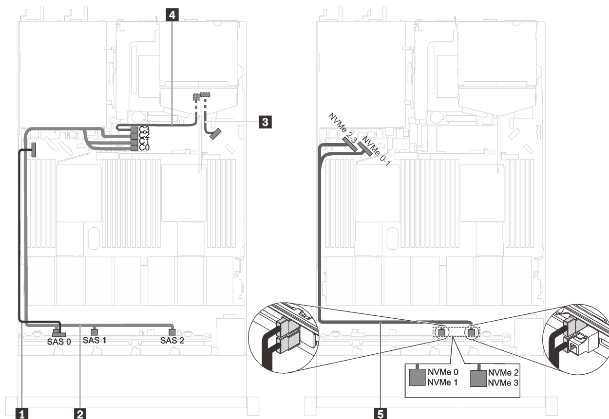
Figura 31. Disposición de los cables para los modelos de servidor con seis unidades SAS/SATA de 2,5 pulgadas, cuatro unidades SAS/SATA/NVMe de 2,5 pulgadas, conjunto de unidad posterior HBA/RAID 16i y un conjunto de unidad posterior
