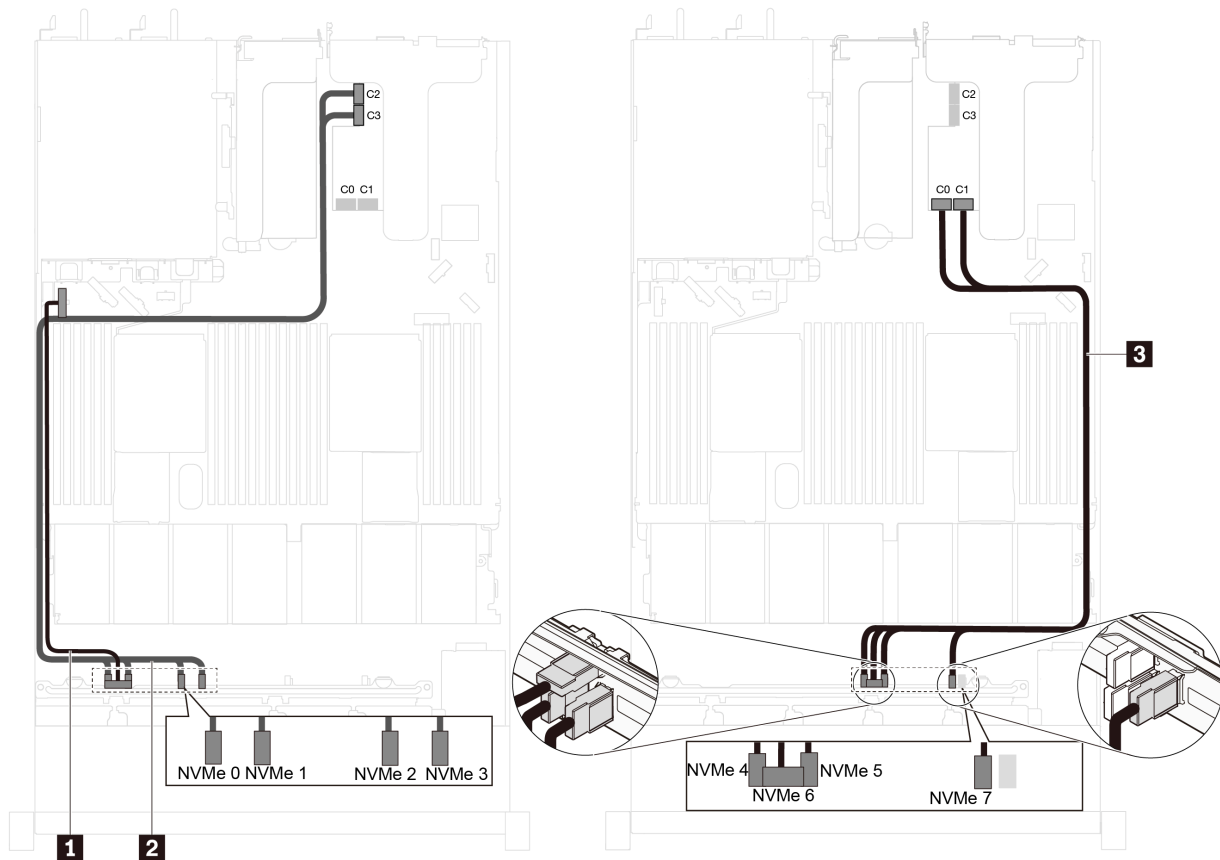
Figura 44. Disposición de cables para modelos de servidor con ocho unidades NVMe de 2,5 pulgadas y un adaptador de conmutador NVMe de 1611-8P en PCIe ranura 2
