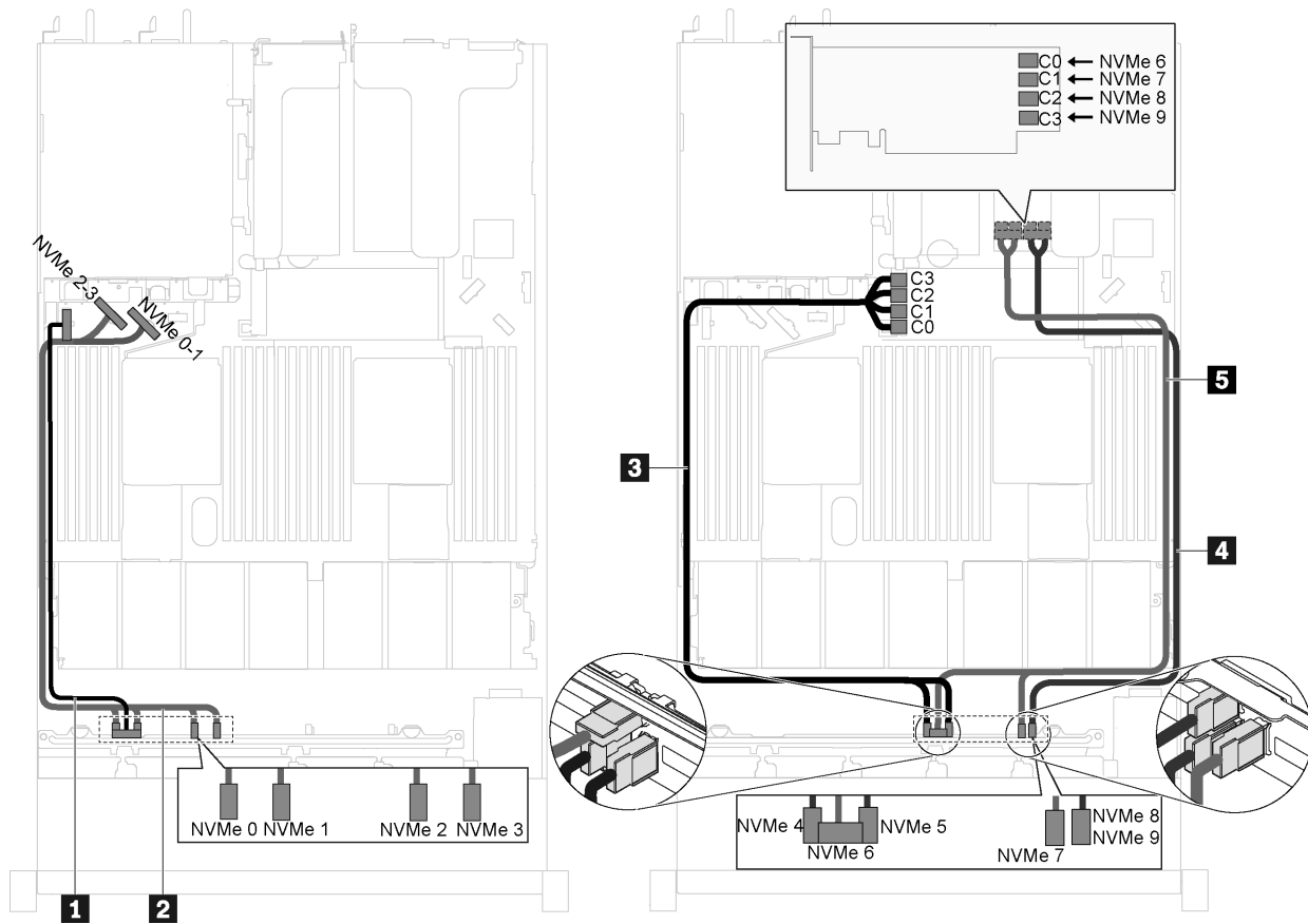
Figura 40. Disposición de cables para modelos de servidor con diez unidades NVMe de 2,5 pulgadas, un adaptador de conmutador NVMe 1610-4P en la ranura de PCIe 2 y un adaptador de conmutador NVMe 810-4P en la ranura de adaptador RAID
