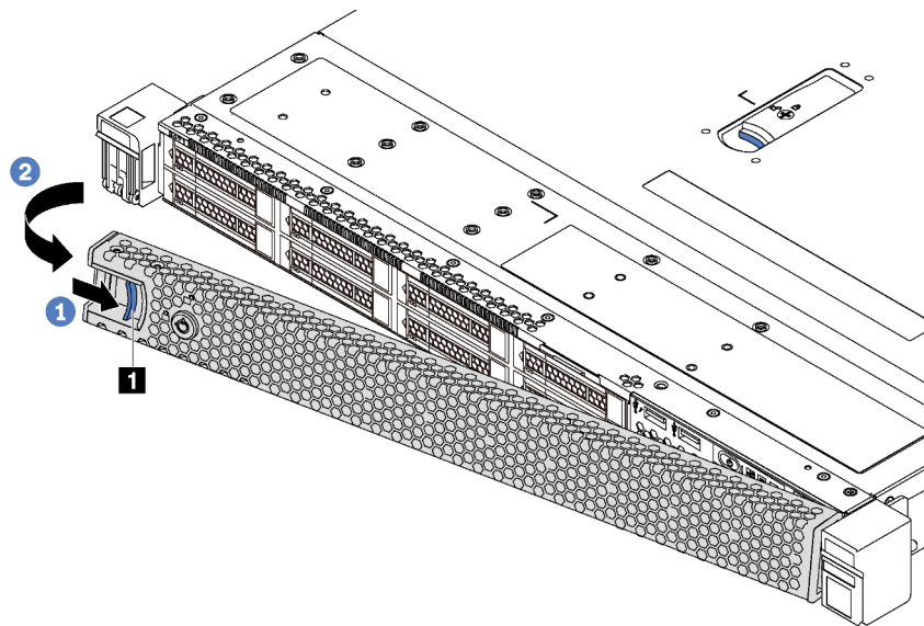
Figura 47. Extracción del marco biselado de seguridad
