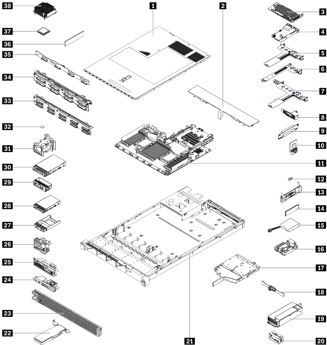
Figura 45. Componentes del servidor
