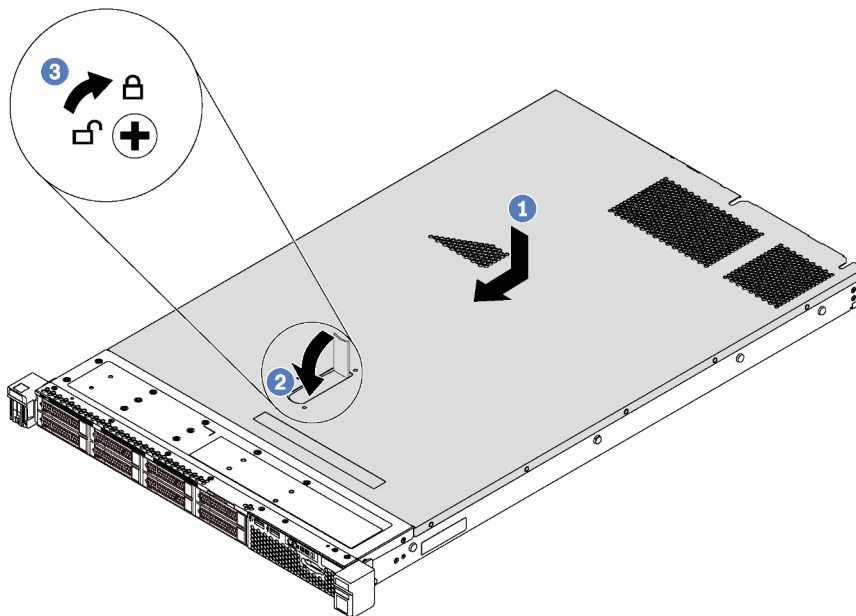
Figura 88. Instalación de la cubierta superior
