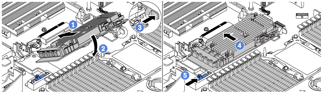
Figura 58. Instalación del adaptador RAID
