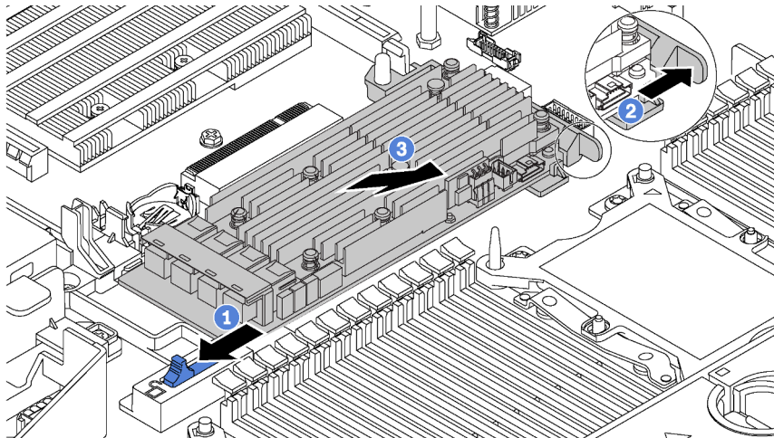
Figura 76. Extracción del adaptador RAID
