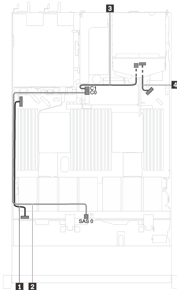
Figura 20. Modelos de servidor con cuatro unidades SAS/SATA de 3,5 pulgadas y conjunto de unidad posterior
