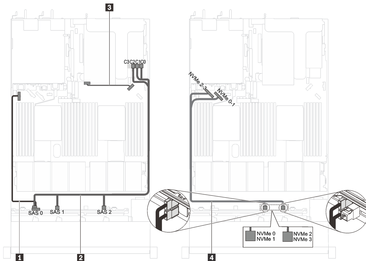
Figura 33. Distribución de cables para modelos de servidor con seis unidades SAS/SATA de 2,5 pulgadas, cuatro unidades SAS/SATA/NVMe de 2,5 pulgadas y una GPU de altura completa y longitud media
