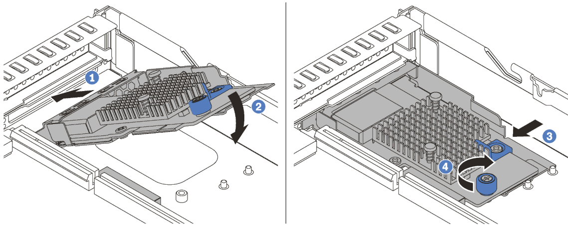
Figura 68. Instalación del adaptador LOM
