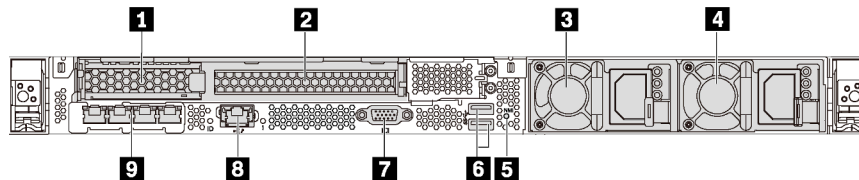
Figura 12. Vista posterior de modelos de servidor con dos ranuras de PCIe
