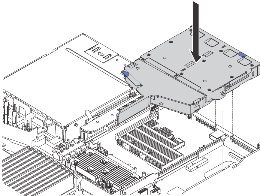
Figura 62. Instalación del conjunto de unidad de intercambio en caliente posterior
