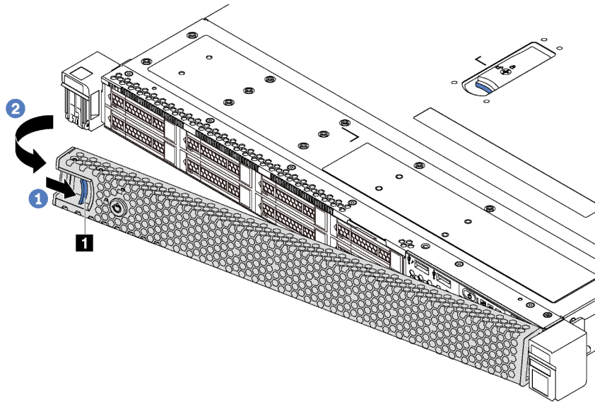
Figure 59. Retrait du panneau de sécurité
