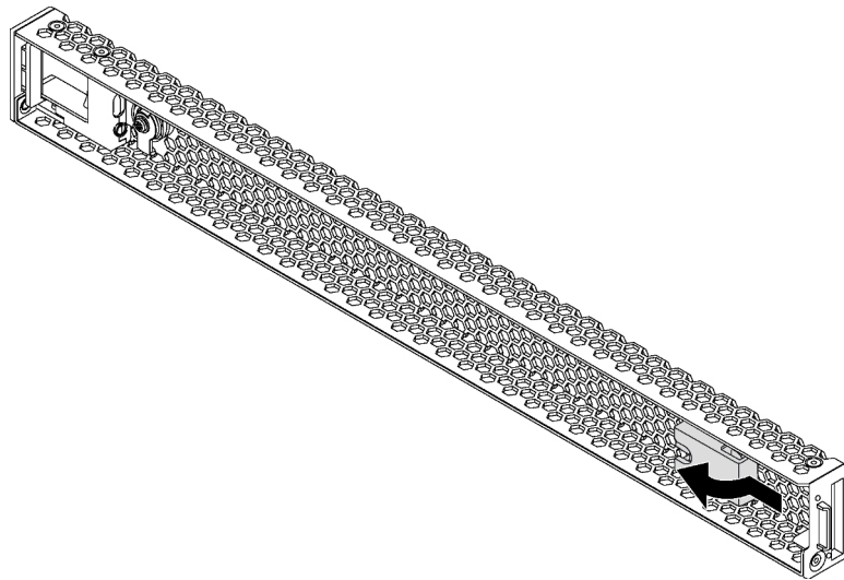
Figure 60. Retrait de la clé
