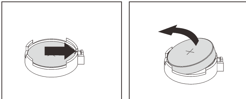
Figure 100. Retrait de la pile CMOS
