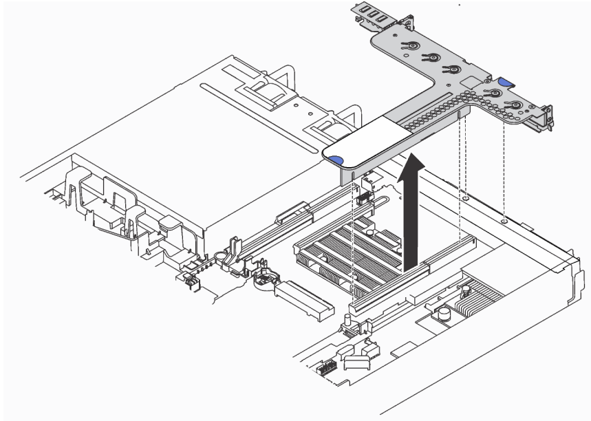
Figure 78. Retrait de l'assemblage de carte mezzanine
