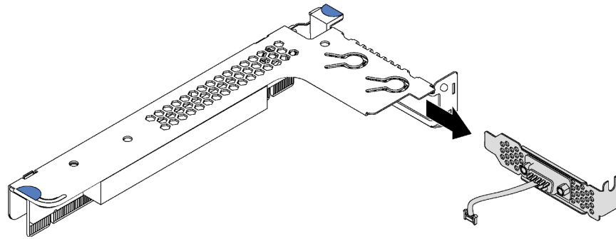
Figure 112. Retrait du module de port série
