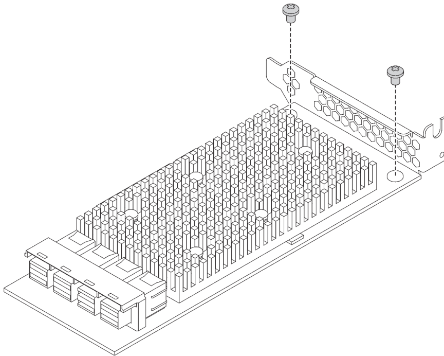
Figure 88. Installation du support extra-plat dans l'adaptateur RAID
