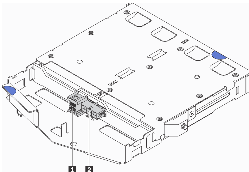
Figure 106. Connecteurs de fond de panier arrière
