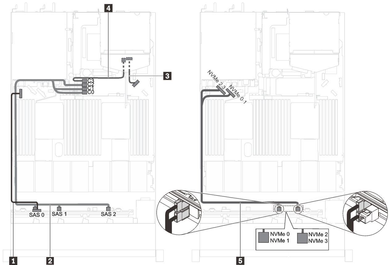
Figure 33. Cheminement des câbles pour modèles de serveur avec six unités SAS/SATA 2,5 pouces, quatre unités SAS/SATA/NVMe 2,5 pouces, un adaptateur RAID/HBA 16i et un bloc d'unités arrière.
