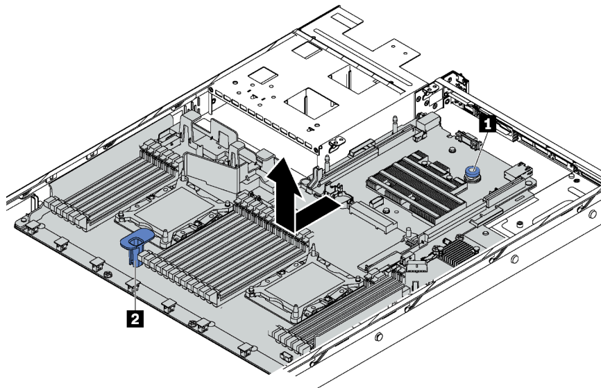
Figure 152. Retrait de la carte mère
