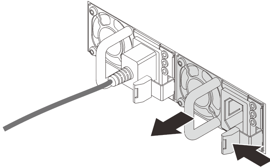
Figure 140. Retrait du bloc d'alimentation remplaçable à chaud
