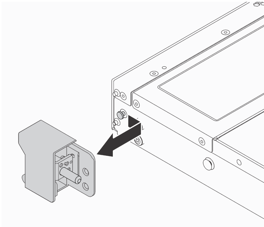
Figure 54. Retrait du taquet d'armoire
