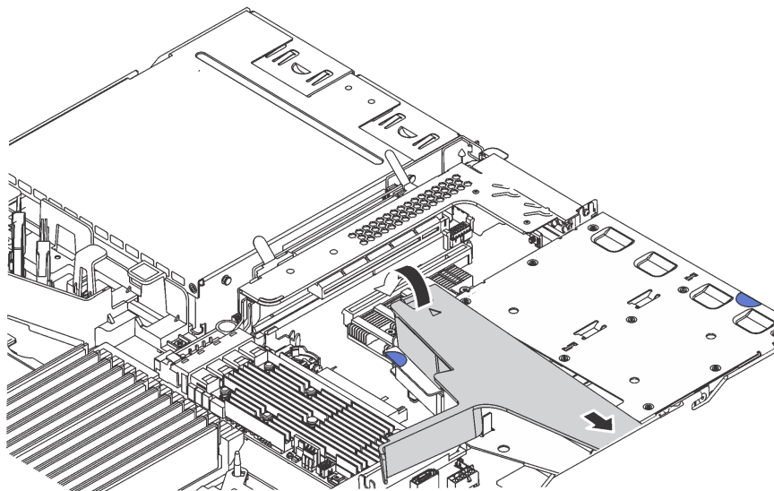
Figure 99. Installation de la grille d'aération
