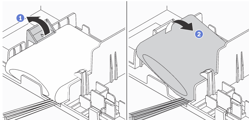
Figure 123. Retrait d'un module de supercondensateur RAID au bas de la grille d'aération
