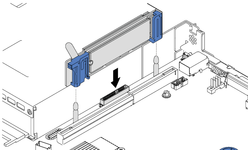
Figure 122. Installation du fond de panier M.2
