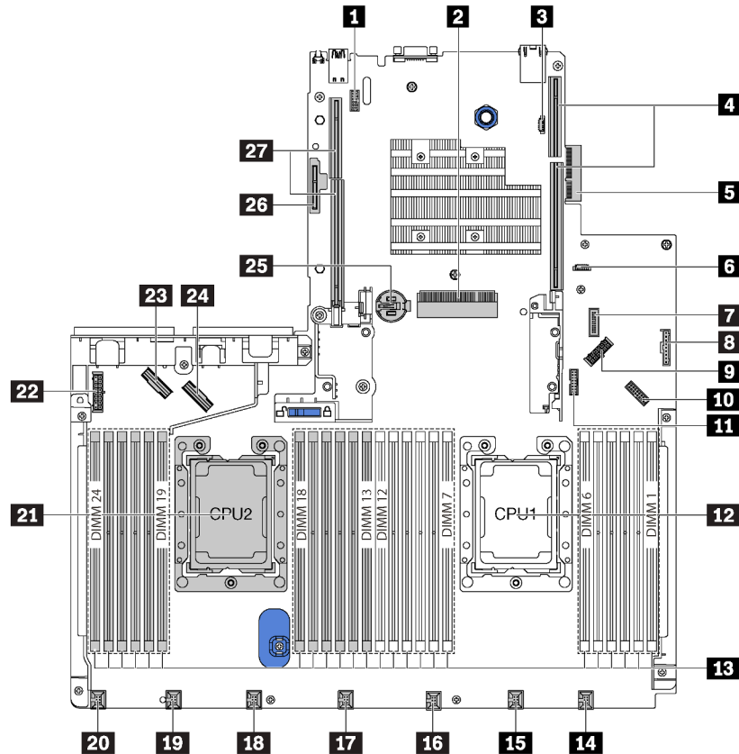
Figure 18. Composants de la carte mère
