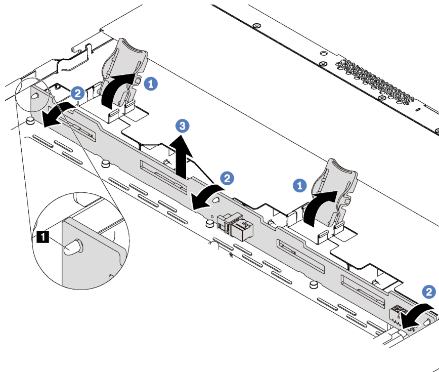
Figure 89. Retrait du fond de panier pour quatre unités remplaçables à chaud 3,5 pouces
