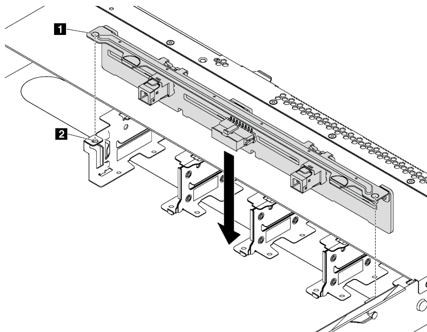
Figure 92. Installation du fond de panier pour huit unités remplaçables à chaud 2,5 pouces
