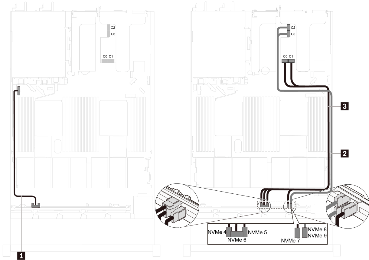
Figure 43. Cheminement des câbles pour les modèles de serveur avec dix unités NVMe 2,5 pouces et un adaptateur de commutateur NVMe 1611-8P dans l'emplacement PCIe 2
