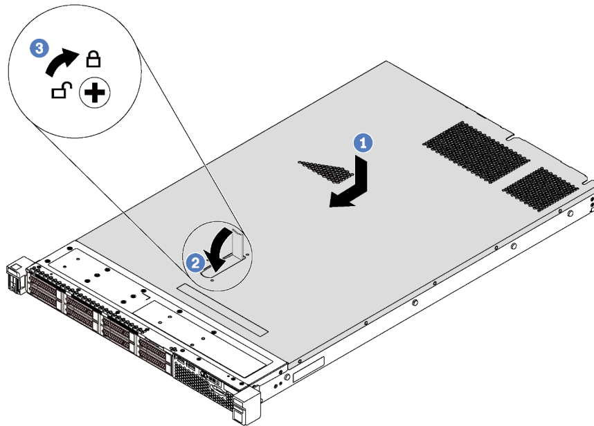
Figure 49. Installation du carter supérieur
