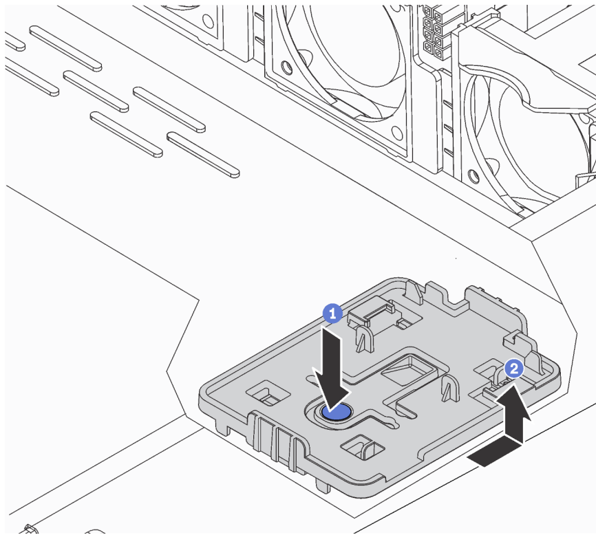
Figure 129. Retrait du plateau
