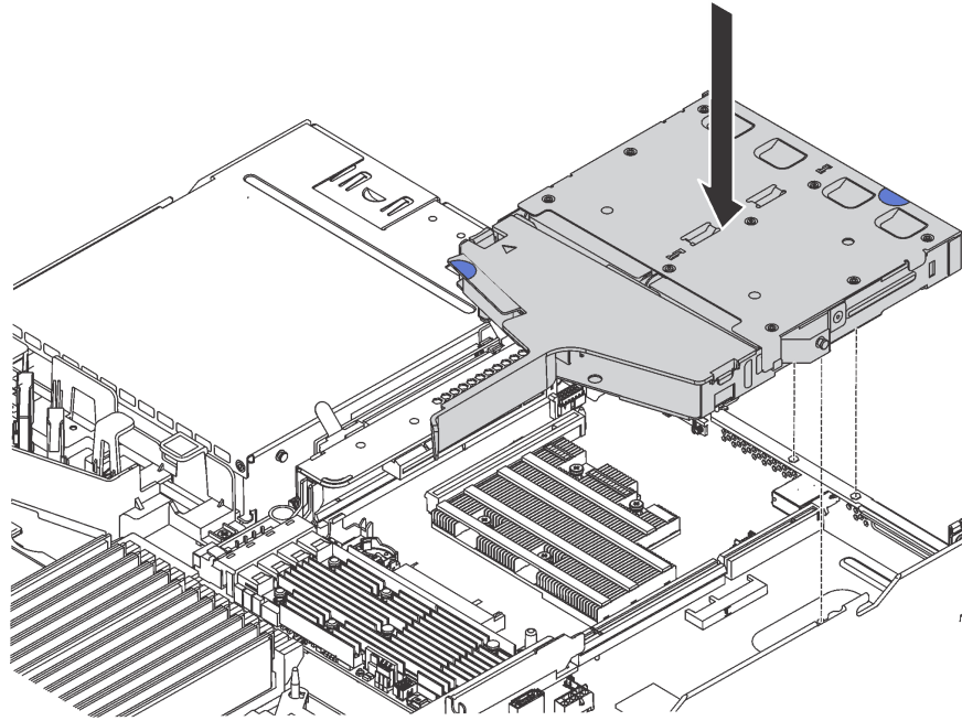
Figure 108. Installation du bloc d'unités remplaçables à chaud arrière
