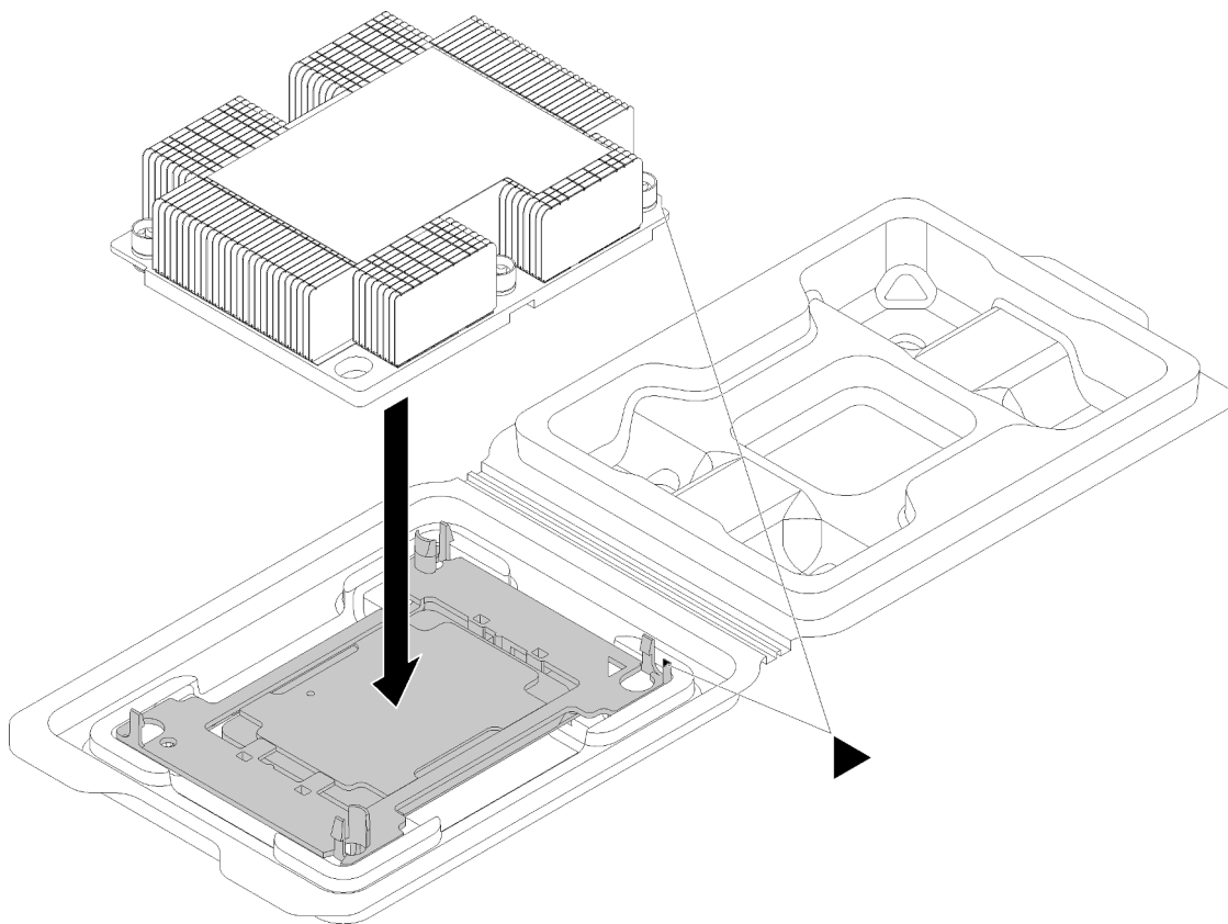
Figure 150. Assembler un module de processeur-dissipateur thermique dans le bac de transport
