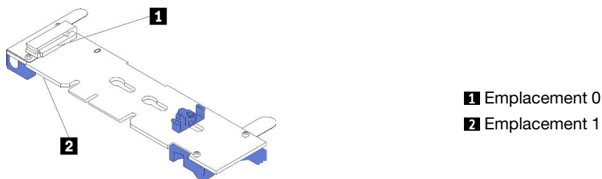
Figure 119. Emplacement de l'unité M.2
