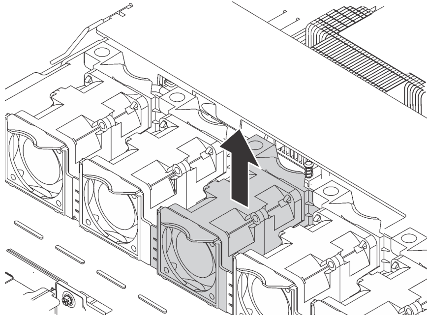
Figure 63. Retrait du ventilateur système
