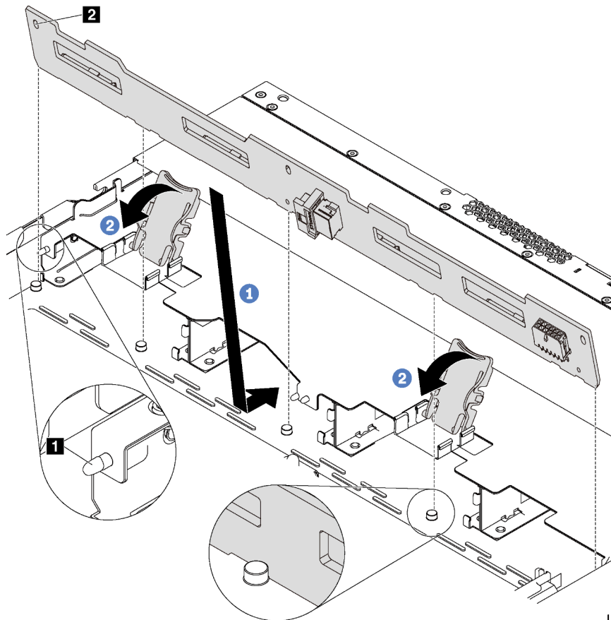
Figure 90. Installation du fond de panier pour quatre unités remplaçables à chaud 3,5 pouces
