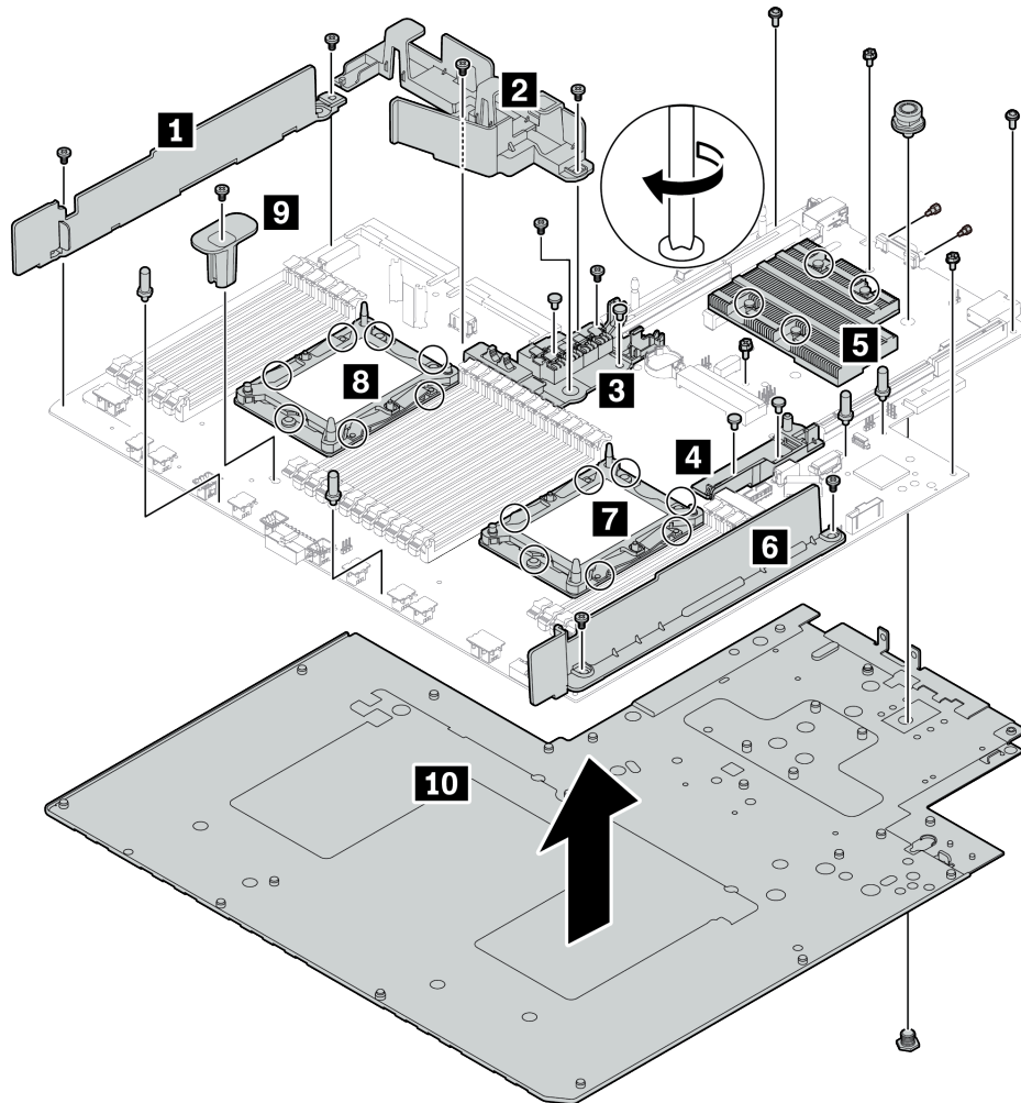
Figure 156. Démontage de la carte mère
