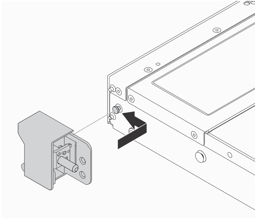
Figure 55. Installation du taquet d'armoire
