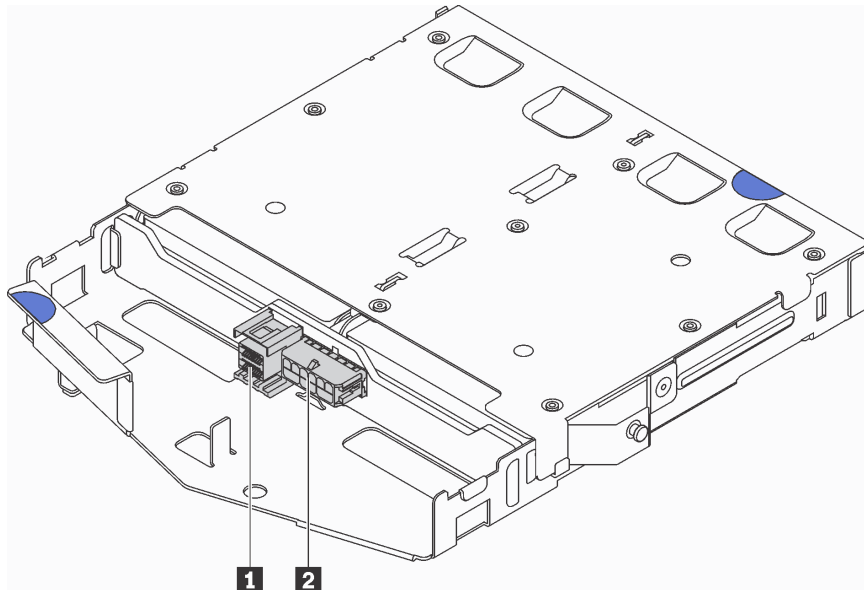
Figure 98. Connecteurs de fond de panier arrière
