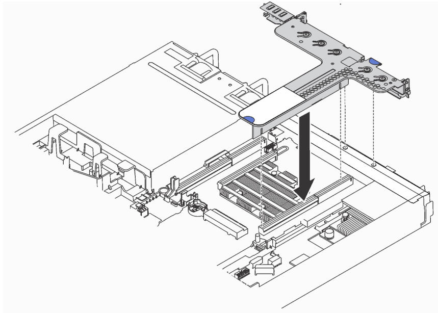
Figure 81. Installation de l'assemblage de cartes mezzanines
