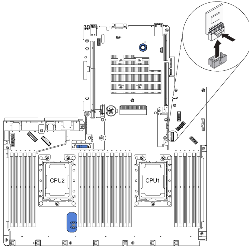
Figure 102. Retrait d'adaptateur TCM/TPM
