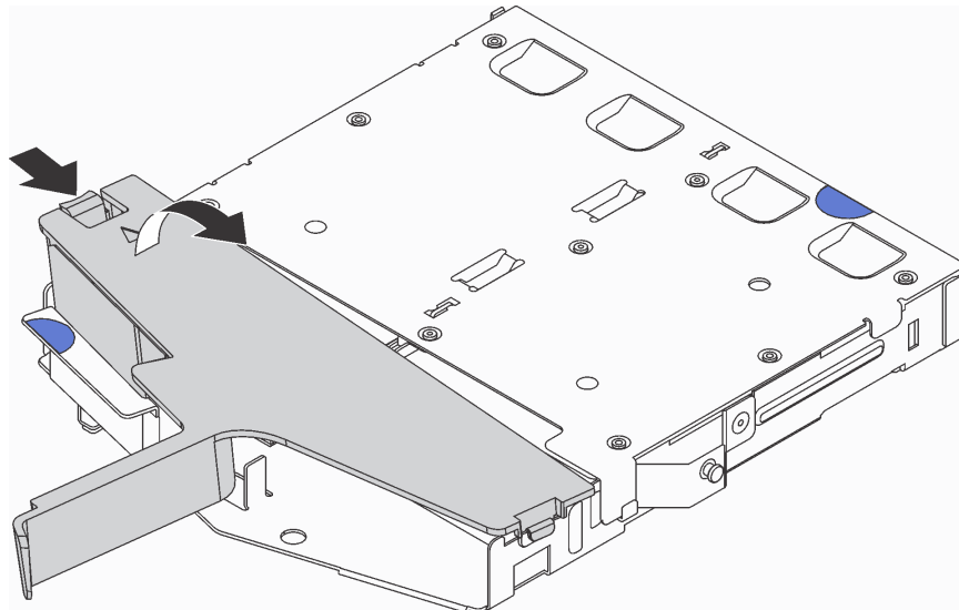
Figure 105. Retrait de la grille d'aération
