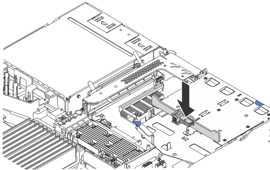
Figure 97. Installation du fond de panier arrière
