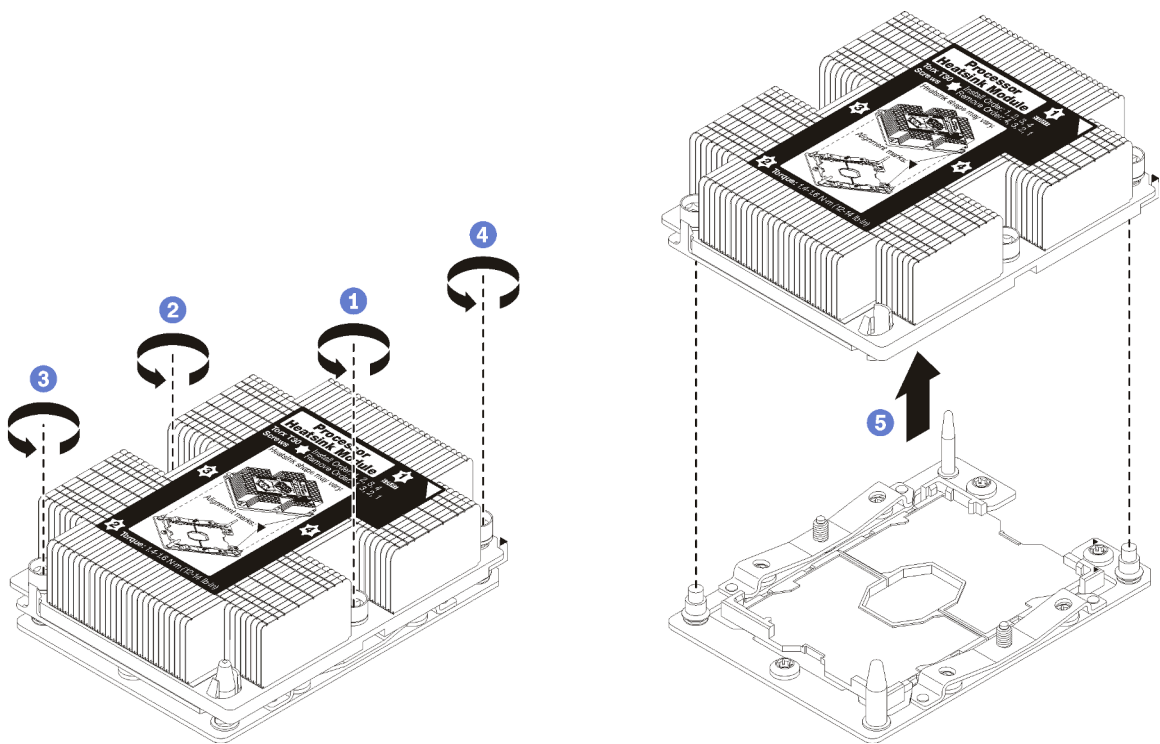
Figure 145. Retrait d'une barrette PHM
