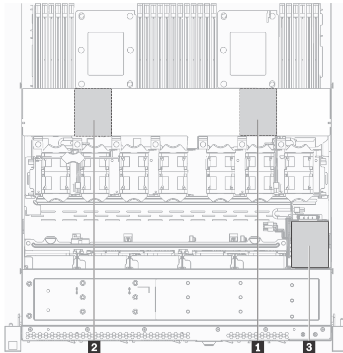
Figure 124. Emplacement du module de supercondensateur RAID
