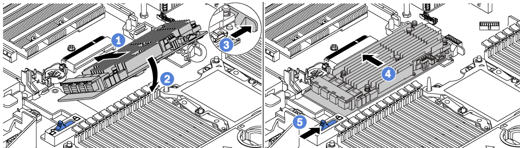
Figure 110. Installation d'adaptateur RAID
