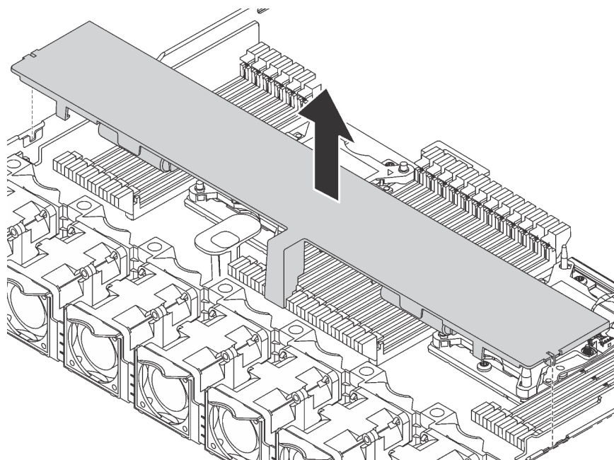
Figure 50. Retrait de la grille d'aération
