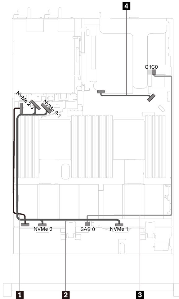
Figure 26. Cheminement des câbles pour les modèles de serveur avec quatre unités SAS/SATA/NVMe 3,5 pouces et une unité GPU pleine hauteur, demi-longueur
