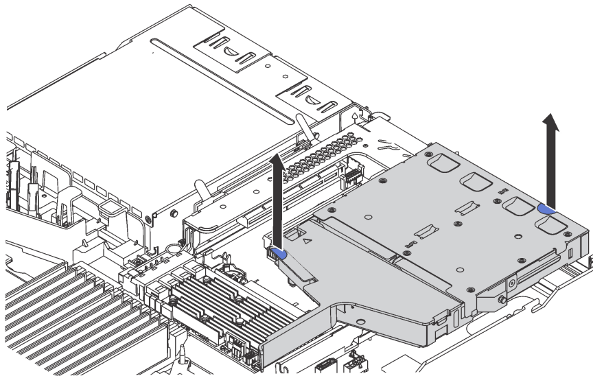
Figure 104. Retrait du bloc d'unités remplaçables à chaud arrière
