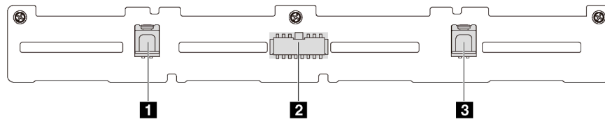
Figure 28. Connecteurs sur le fond de panier pour huit unités SAS/SATA 2,5 pouces
