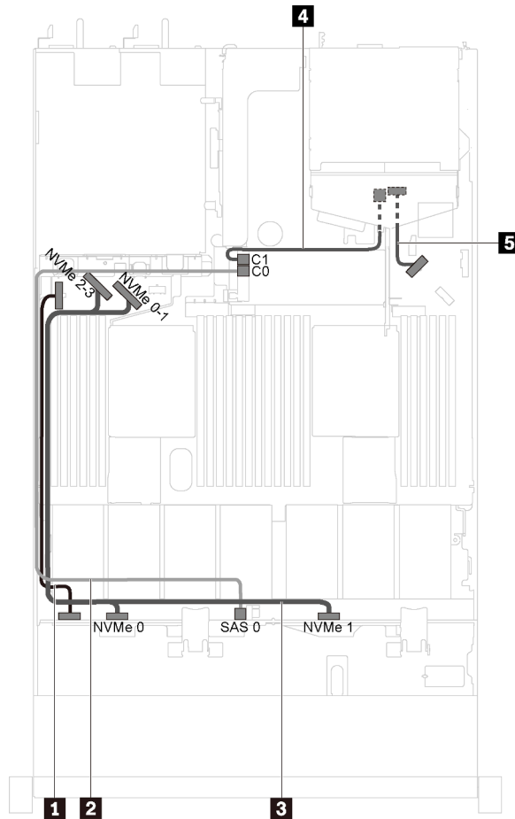
Figure 25. Cheminement des câbles pour les modèles de serveur avec quatre unités SAS/SATA/NVMe 3,5 pouces et un assemblage d'unité arrière
