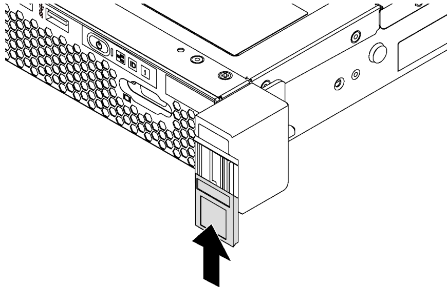
Figure 57. Installation de la plaque d'étiquette d'identification
