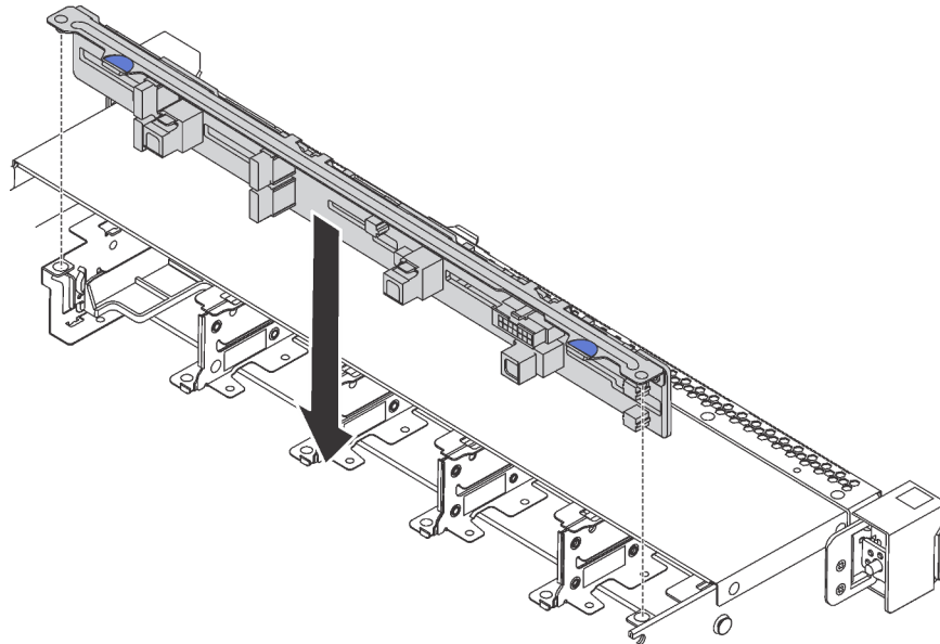
Figure 94. Installation du fond de panier pour dix unités remplaçables à chaud 2,5 pouces
