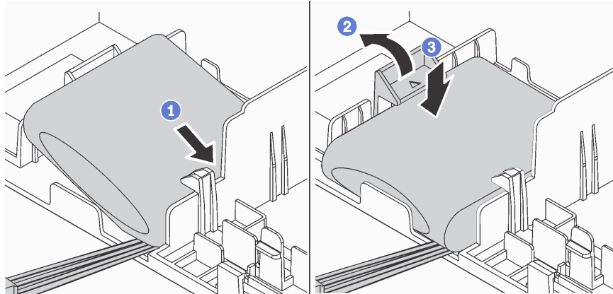
Figure 125. Installer un module de supercondensateur RAID au bas de la grille d'aération
