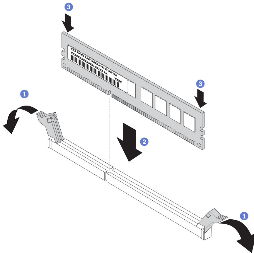
Figure 68. Installation du module de mémoire
