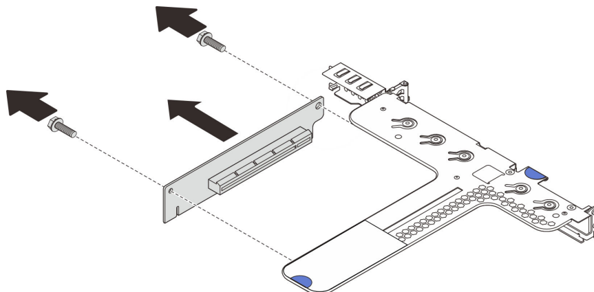
Figure 79. Retrait de la carte mezzanine
