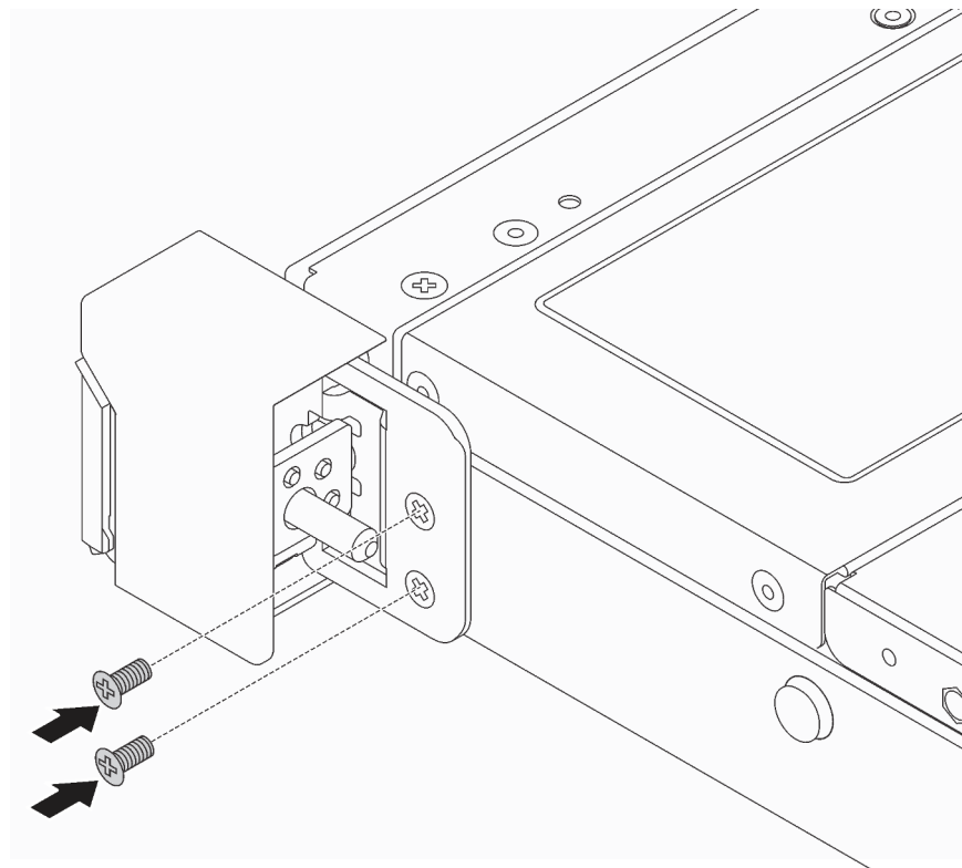
Figure 56. Installation des vis du taquet d'armoire
