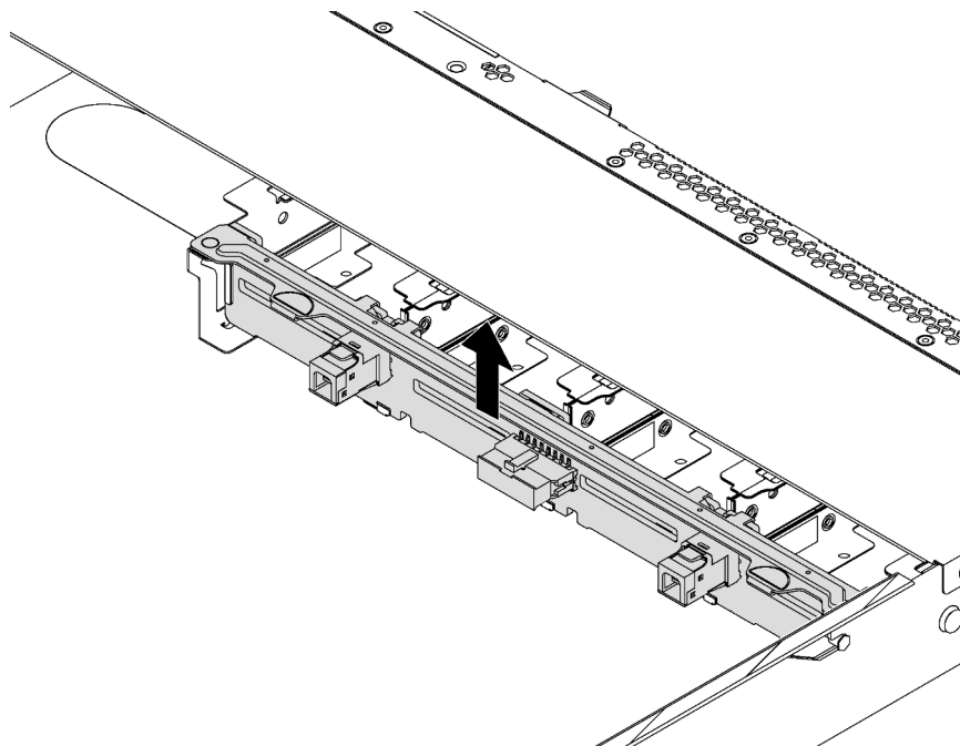
Figure 91. Retrait du fond de panier pour huit unités remplaçables à chaud 2,5 pouces
