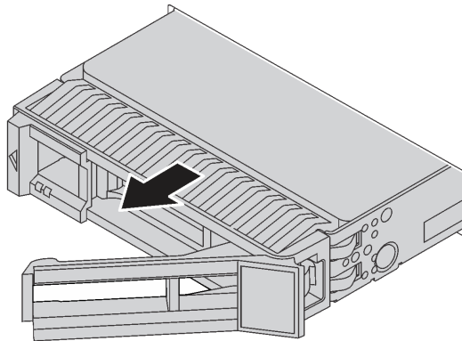
Figure 70. Retrait de l'unité remplaçable à chaud
