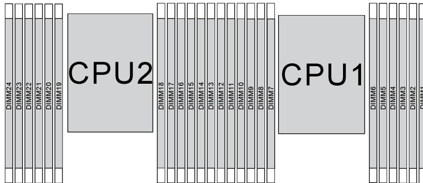
Figure 67. emplacements de module de mémoire sur la carte mère
