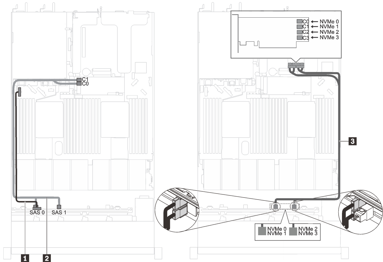
Figure 36. Cheminement des câbles pour modèles de serveur avec six unités SAS/SATA 2,5 pouces, quatre unités NVMe 2,5 pouces, un adaptateur RAID/HBA 8i et un adaptateur de commutateur NVMe 1610-4P dans l'emplacement PCIe 2
