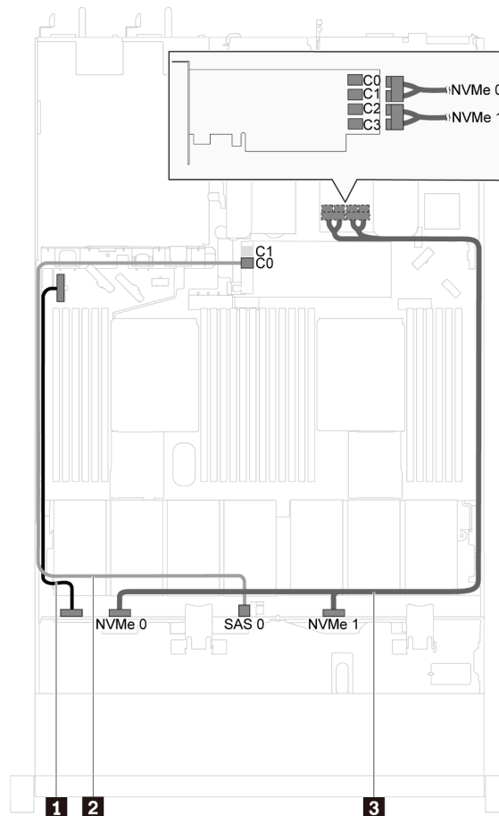
Figure 27. Cheminement des câbles pour les modèles de serveur avec quatre unités SAS/SATA/NVMe 3,5 pouces et un adaptateur de commutateur NVMe 1610-4P dans l'emplacement PCIe 2
