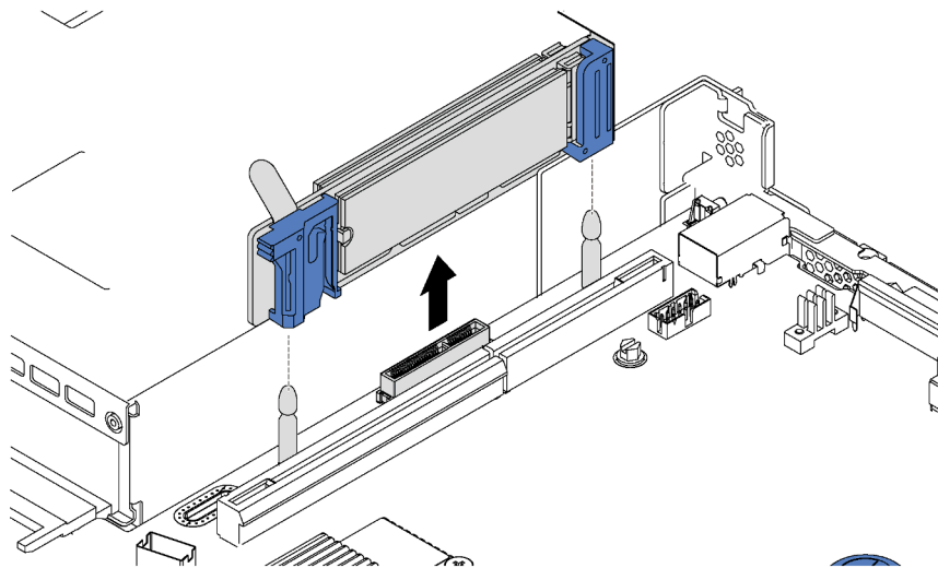
Figure 116. Retrait du fond de panier M.2
