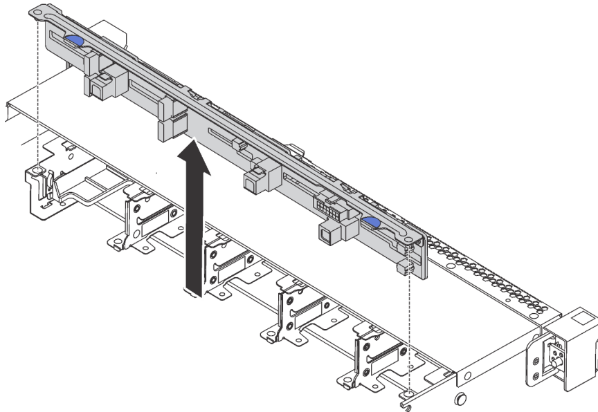
Figure 93. Retrait du fond de panier pour dix unités remplaçables à chaud 2,5 pouces
