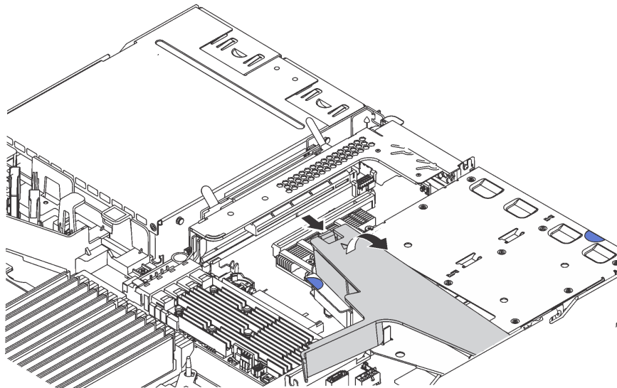
Figure 95. Retrait de la grille d'aération
