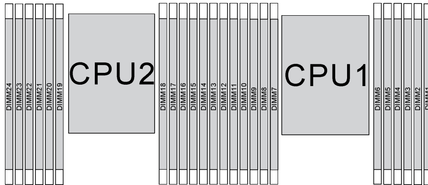
Figure 66. emplacements de module de mémoire sur la carte mère
