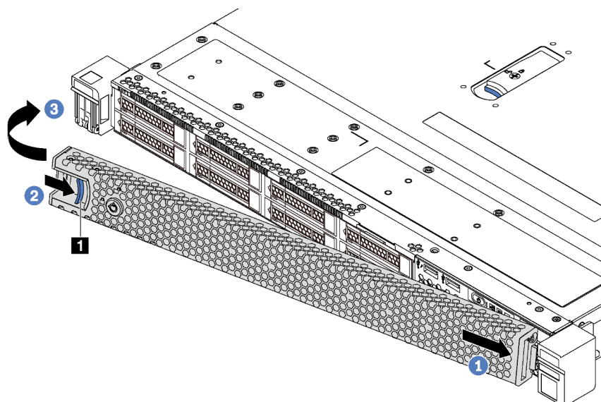
Figure 61. Installation du panneau de sécurité
