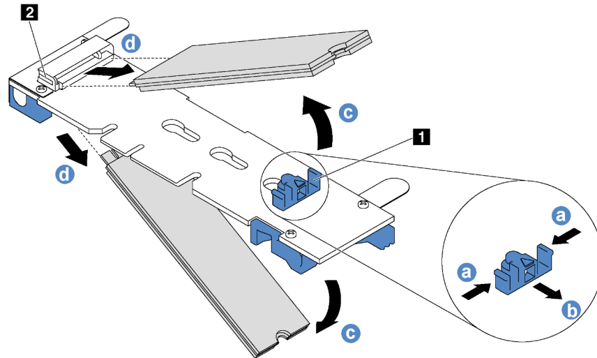
Figure 117. Retrait d'une unité M.2
