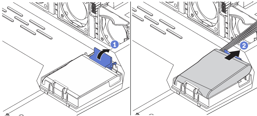
Figure 126. Retrait du module de supercondensateur RAID du châssis
