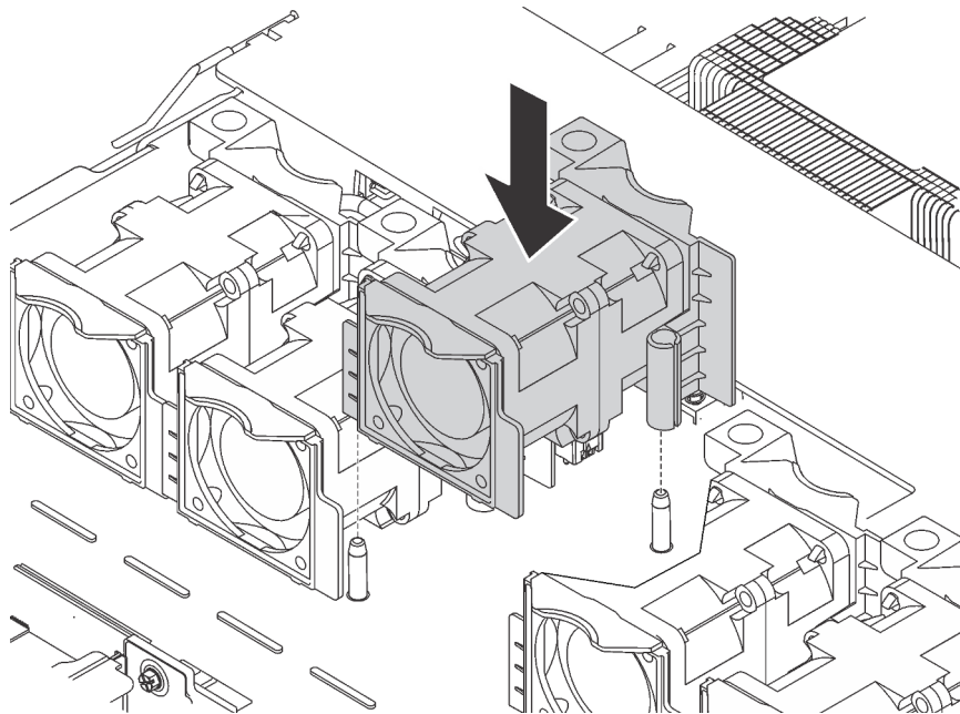
Figure 64. Installation du ventilateur système
