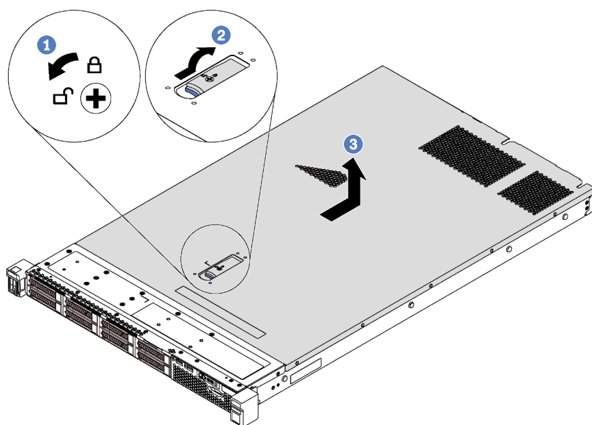
Figure 48. Retrait du carter supérieur
