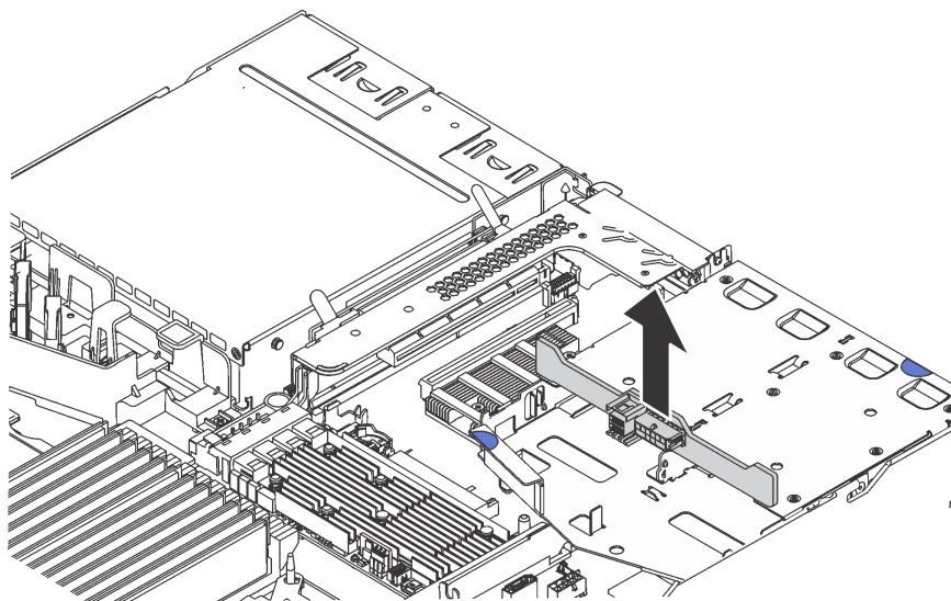
Figure 96. Retrait du fond de panier arrière
