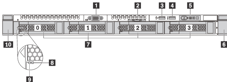
Figure 7. Vue avant des modèles de serveur équipés de quatre baies d'unité 3,5 pouces
