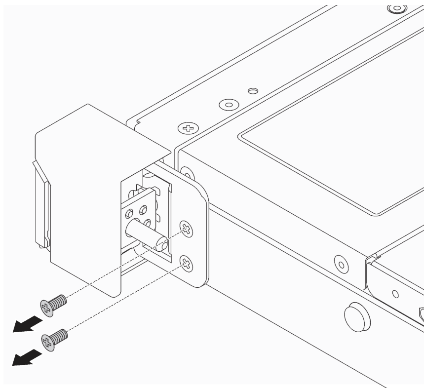
Figure 53. Retrait des vis du taquet d'armoire
