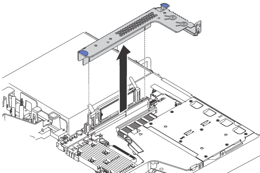
Figure 113. Retrait de l'assemblage de carte mezzanine
