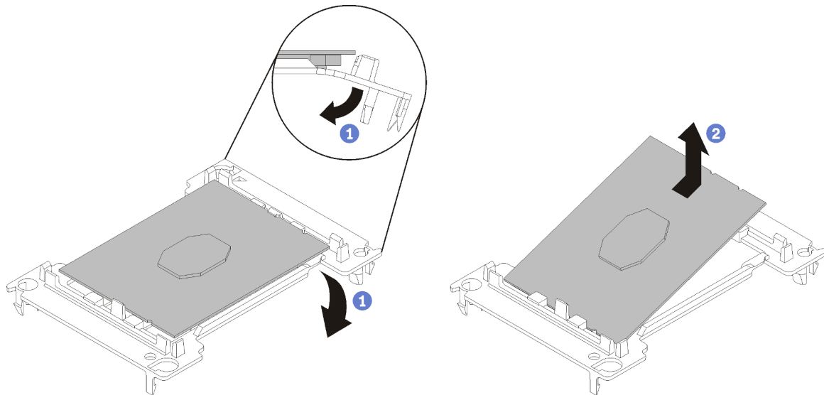
Figure 147. Retrait de la patte de maintien d'un processeur
