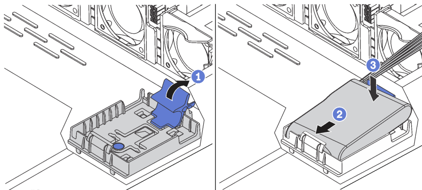
Figure 131. Installation du module de supercondensateur RAID dans le châssis
