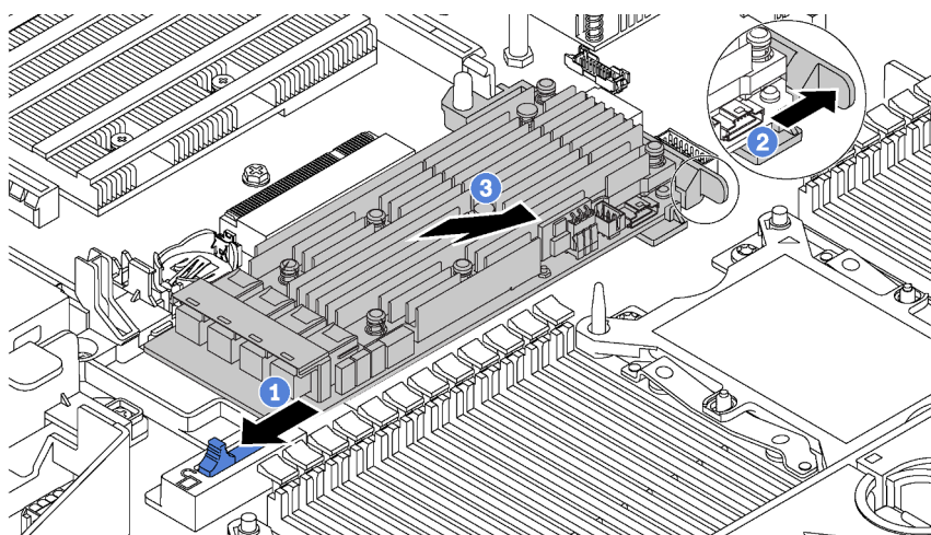
Figure 109. Retrait d'adaptateur RAID
