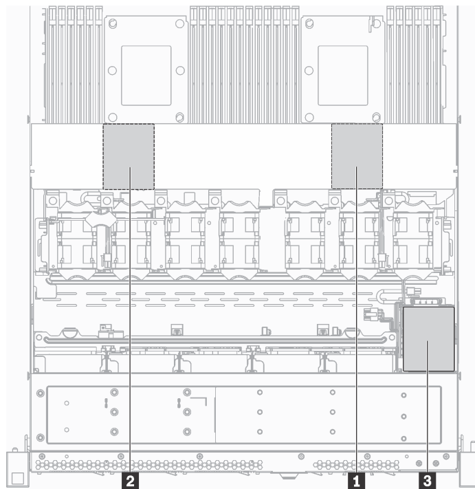
Figure 128. Emplacement du module de supercondensateur RAID
