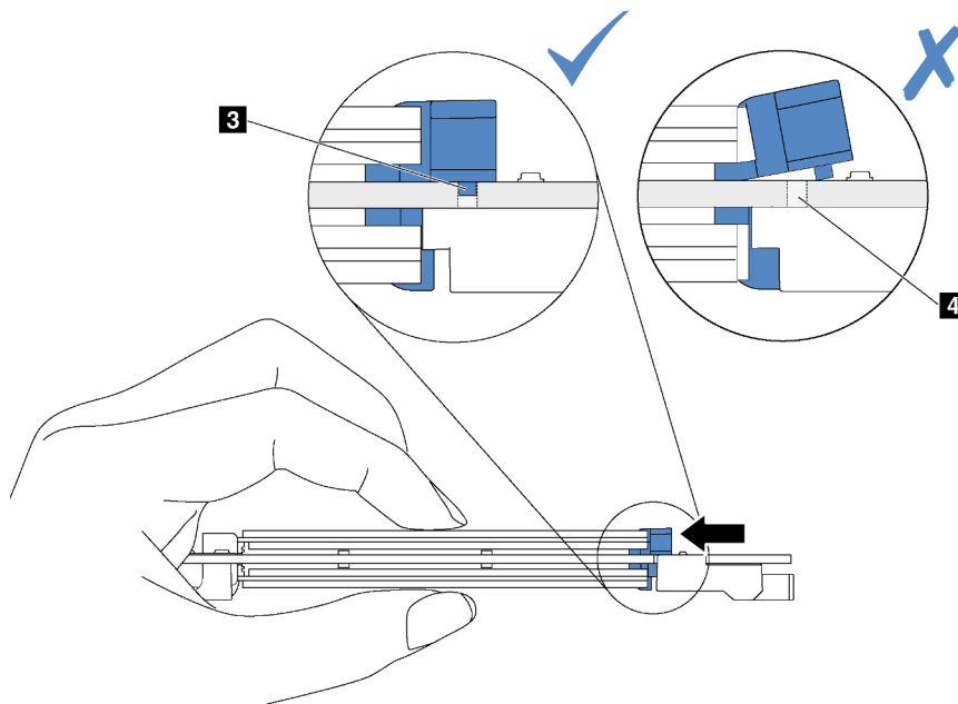
Figure 121. Instruction pour faire glisser la patte
