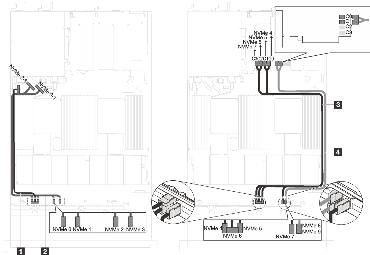
Figure 41. Cheminement des câbles pour les modèles de serveur à dix unités NVMe 2,5 pouces, un adaptateur de commutateur NVMe 1610-4P dans l'emplacement PCIe 2 et un adaptateur de commutateur NVMe 1610-4P dans l'emplacement PCIe 3
