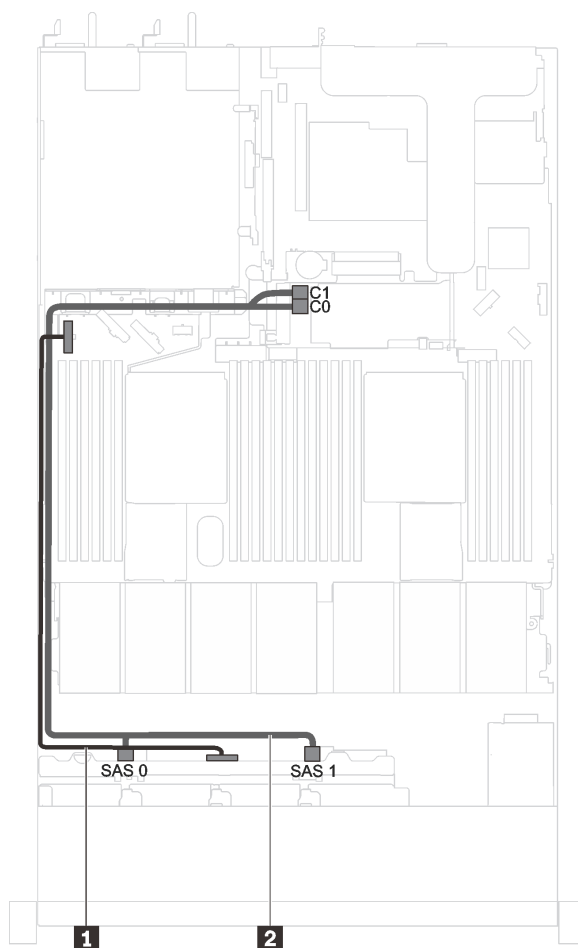
Figure 29. Cheminement des câbles pour modèles de serveur avec huit unités SAS/SATA 2,5 pouces et un adaptateur RAID/HBA 8i
