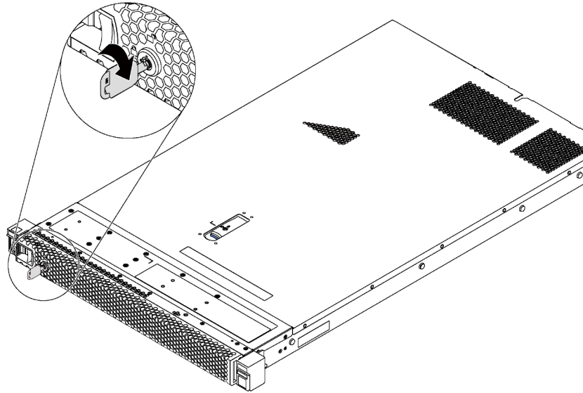
Figure 58. Déverrouillage du panneau de sécurité
