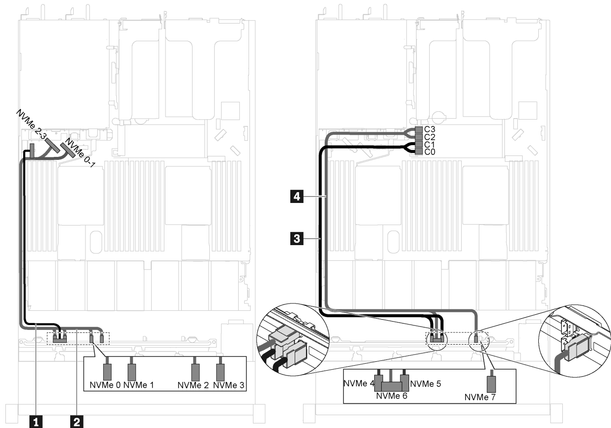
Figure 44. Cheminement des câbles pour les modèles de serveur avec huit unités NVMe 2,5 pouces et un adaptateur de commutateur NVMe 810-4P dans l'emplacement de l'adaptateur RAID
