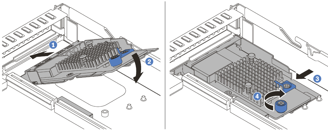
Figure 74. Installation d'adaptateur LOM
