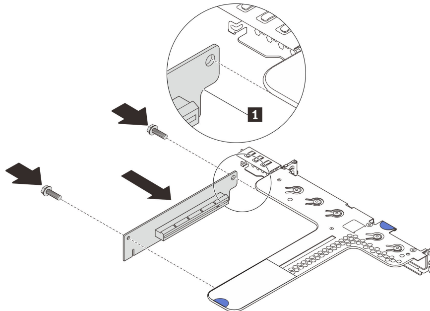
Figure 80. Installation d'une carte mezzanine
