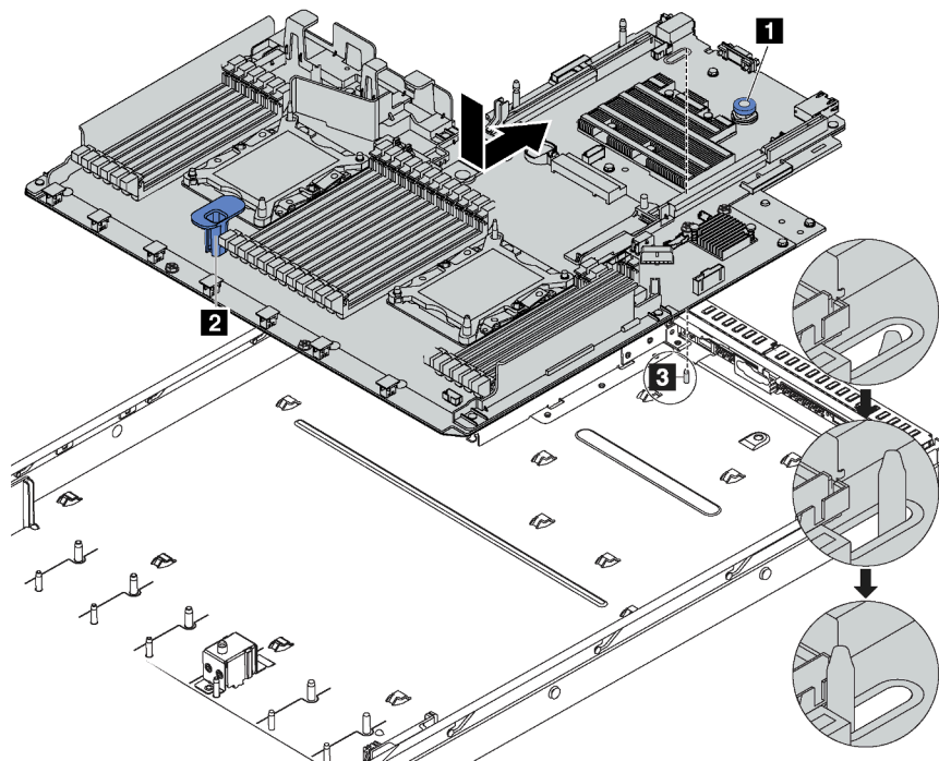
Figure 153. Installation de la carte mère
