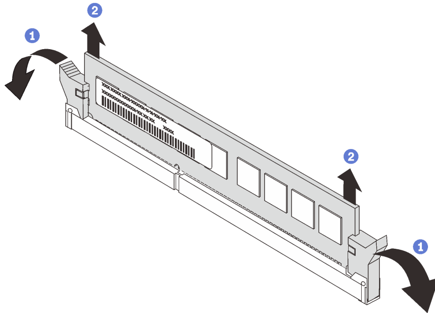
Figure 65. Retrait d'un module de mémoire
