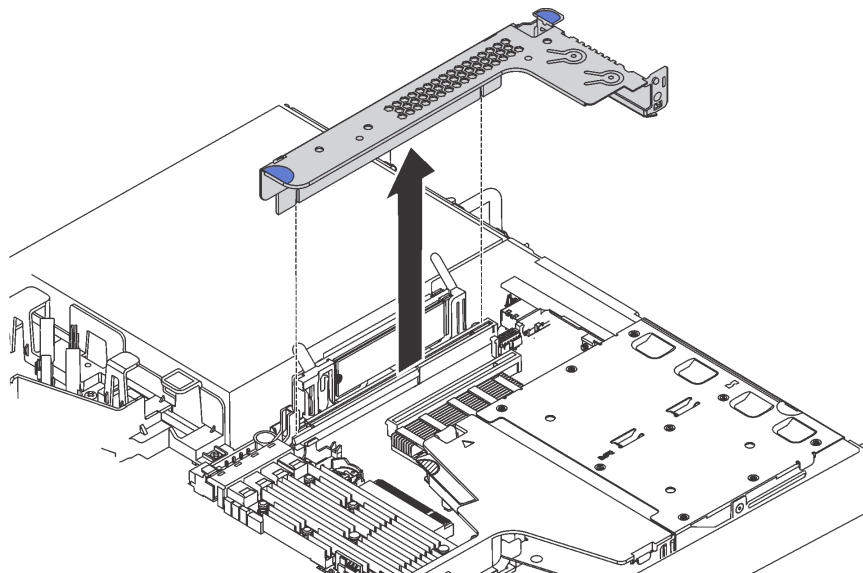
Figure 111. Retrait de l'assemblage de carte mezzanine
