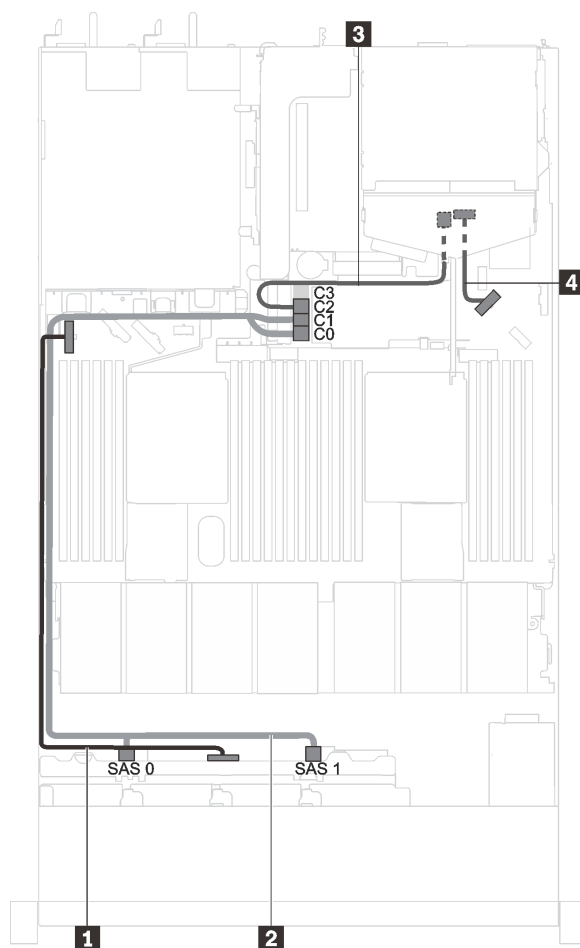
Figure 30. Cheminement des câbles pour modèles de serveur avec huit unités SAS/SATA 2,5 pouces, un adaptateur RAID/HBA 16i et un bloc d'unités arrière
