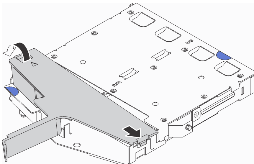
Figure 107. Installation de la grille d'aération
