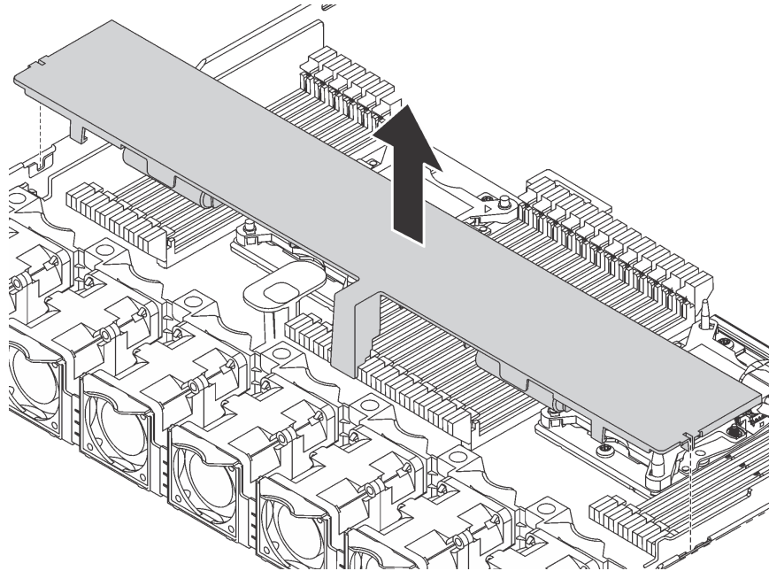
그림 49. 공기 조절 장치 제거
