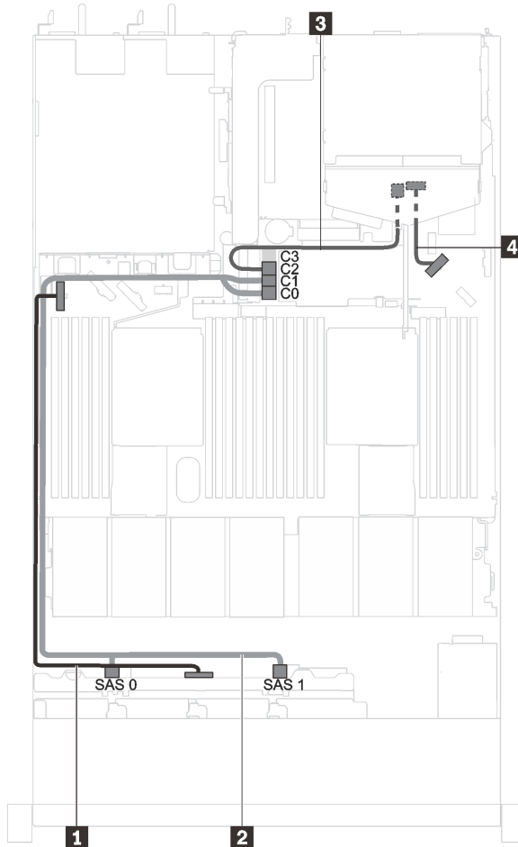
그림 28. 2.5인치 SAS/SATA 드라이브 8개, 16i HBA/RAID 어댑터 1개 및 뒷면 드라이브 어셈블리가 지원되는 서버 모델의 케이블 배선
