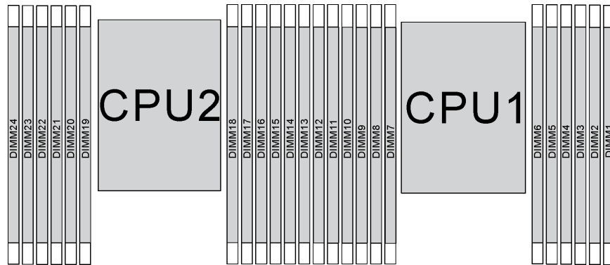
그림 54. 시스템 보드의 메모리 모듈 슬롯
