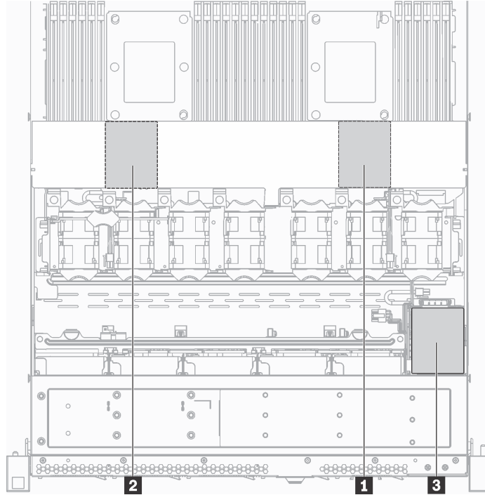
그림 81. RAID 슈퍼 캐패시터 모듈 위치
