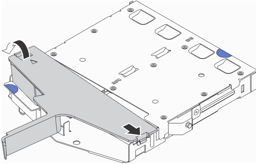
그림 61. 공기 조절 장치 설치
