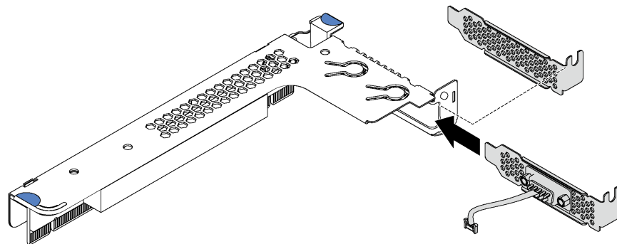
그림 79. 직렬 포트 모듈 설치
