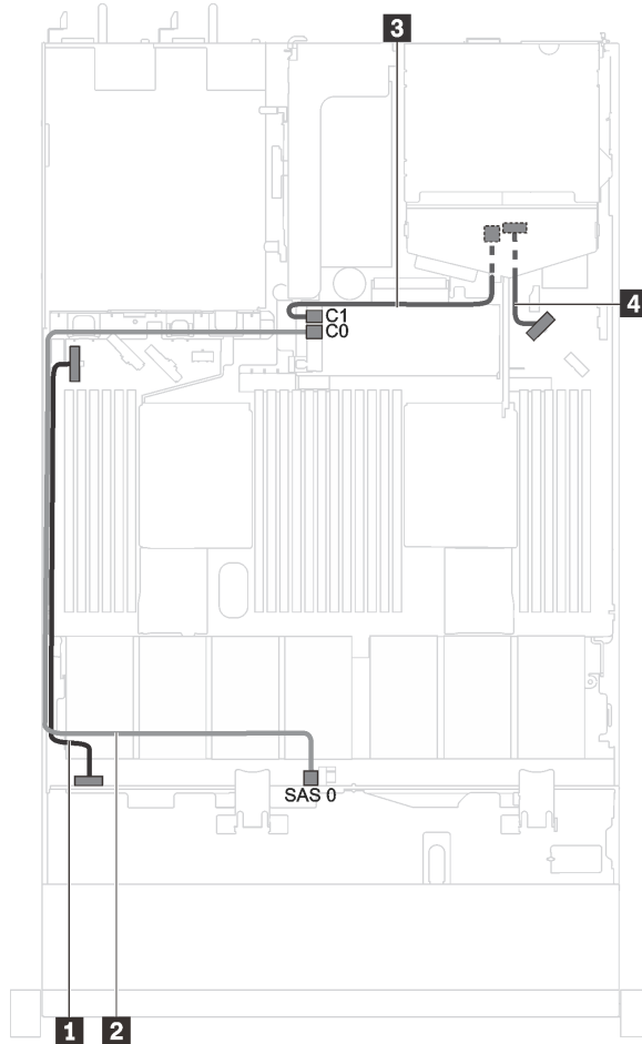
그림 20. 4개의 3.5인치 SAS/SATA 드라이브 및 뒷면 드라이브 어셈블리가 지원되는 서버 모델
