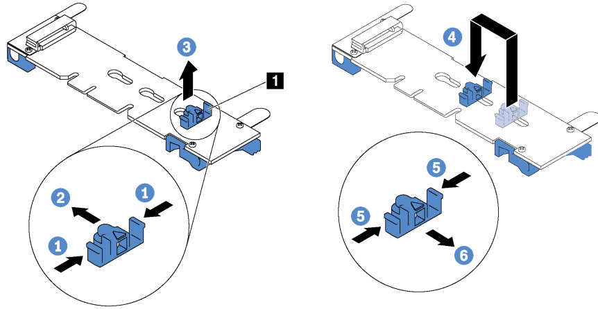
그림 67. M.2 고정장치 조정
