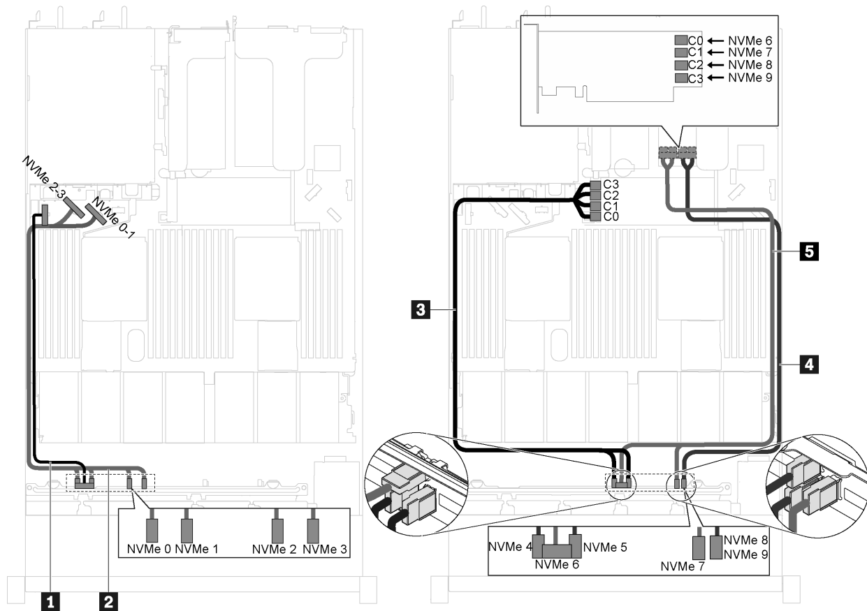
그림 40. 10개의 2.5인치 NVMe 드라이브, PCIe 슬롯 2에 1개의 1610-4P NVMe 스위치 어댑터 및 RAID 어댑터 슬롯에 1개의 810-4P NVMe 스위치 어댑터가 있는 서버 모델의 케이블 배선
