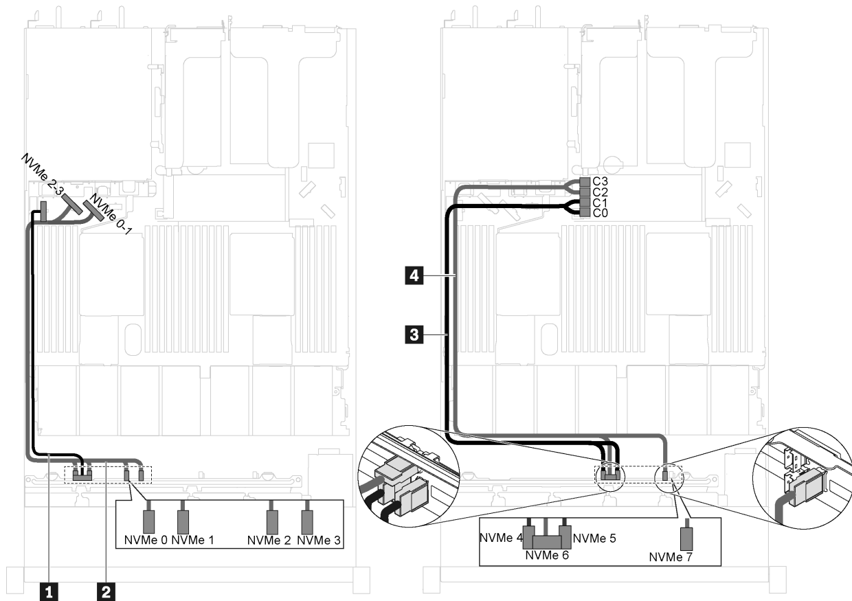
그림 42. 8개의 2.5인치 NVMe 드라이브 및 RAID 어댑터 슬롯에 1개의 810-4P NVMe 스위치 어댑터가 있는 서버 모델의 케이블 배선
