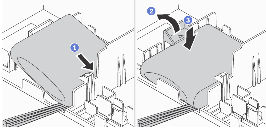
그림 82. 공기 조절 장치의 맨 아래에 RAID 슈퍼 커패시터 모듈 설치
