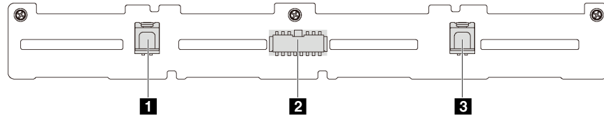
그림 26. 8개의 2.5인치 SAS/SATA 드라이브용 백플레인의 커넥터
