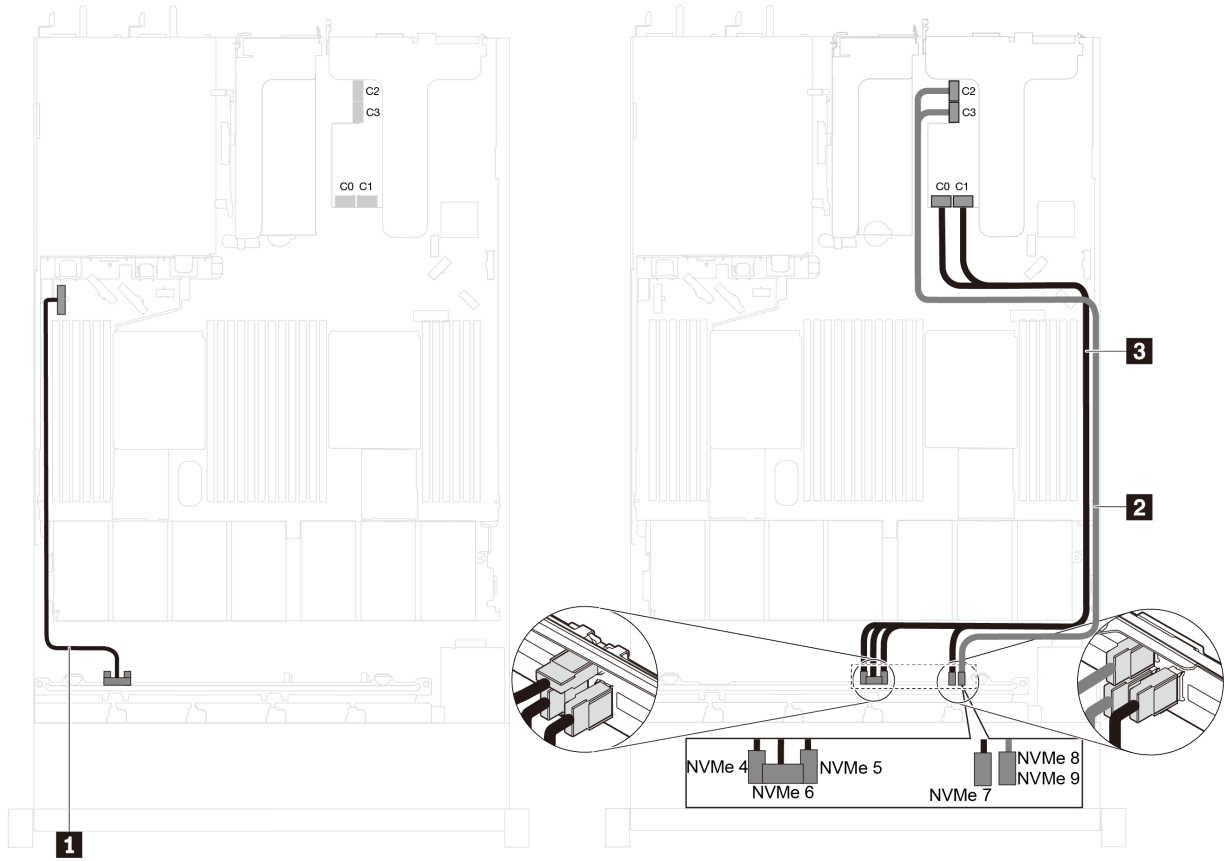
그림 41. PCIe 슬롯 2에 2.5인치 NVMe 드라이브 10개 및 1611-8P NVMe 스위치 어댑터 1개를 장착한 서버 모델의 케이블 배선
