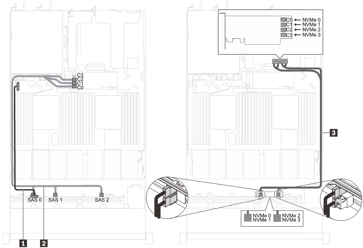
그림 36. 2.5인치 SAS/SATA 드라이브 6개, 2.5인치 NVMe 드라이브 4개, 16i HBA/RAID 어댑터 1개 및 PCIe 슬롯 2에 1610-4P NVMe 스위치 어댑터 1개가 지원되는 서버 모델의 케이블 배선
