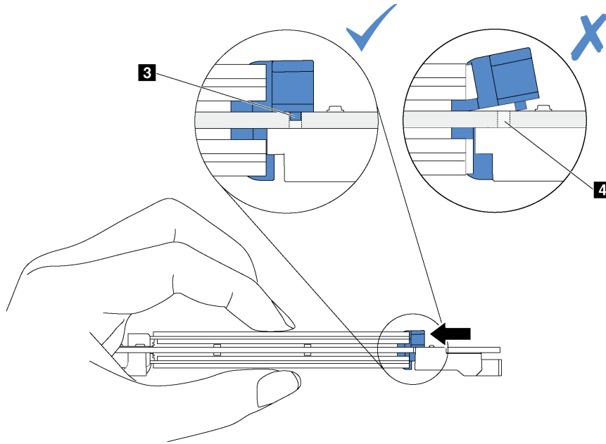
그림 65. 고정장치를 미는 방법
