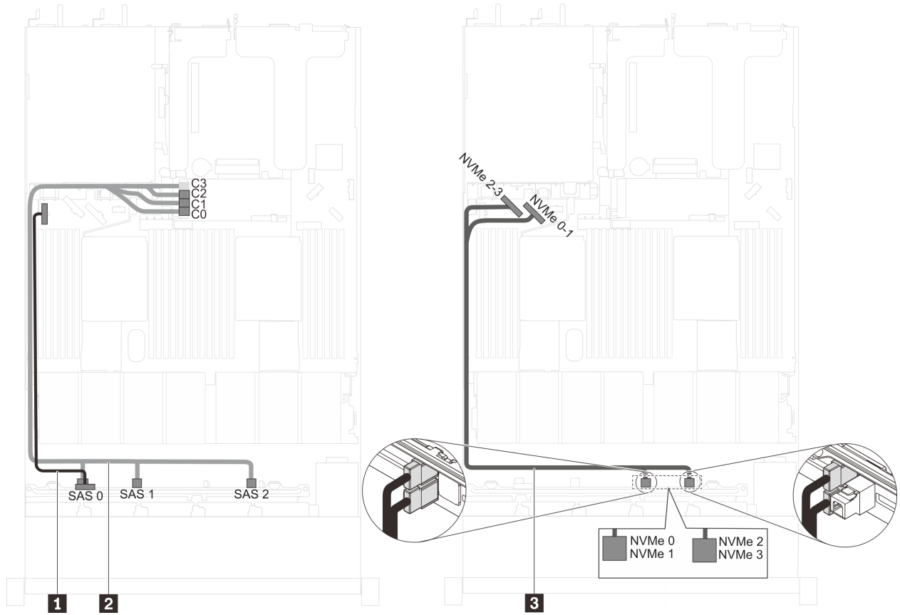
그림 35. Intel Xeon 6154, 6254 및 6240Y 프로세서, 2.5인치 SAS/SATA/NVMe 드라이브 4개 및 16i HBA/RAID 어댑터 1개가 지원되는 서버 모델의 케이블 배선
