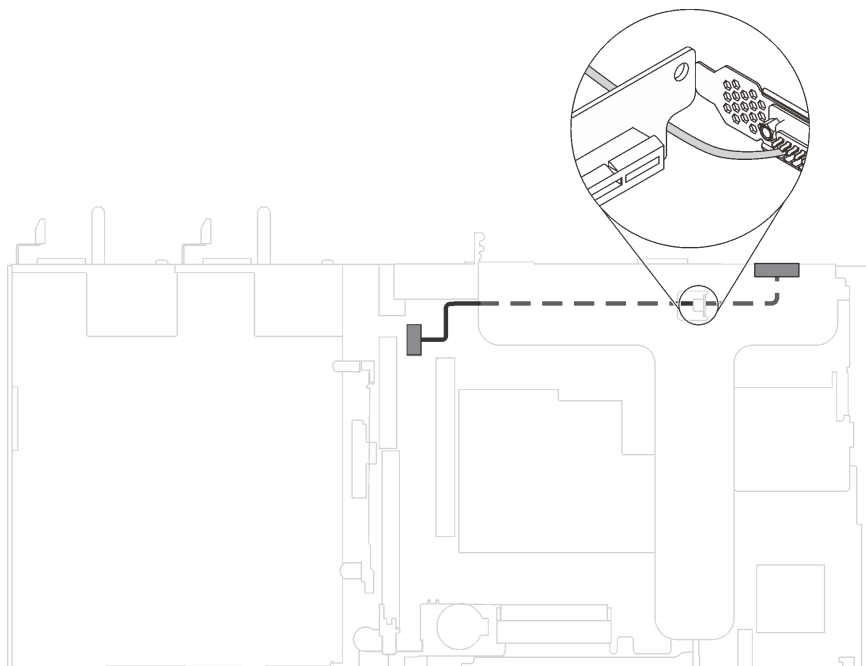
그림 80. PCIe 슬롯 10에 설치된 직렬 포트 모듈의 케이블 라우팅
