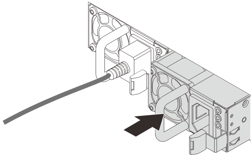
그림 57. 핫 스왑 전원 공급 장치 설치
