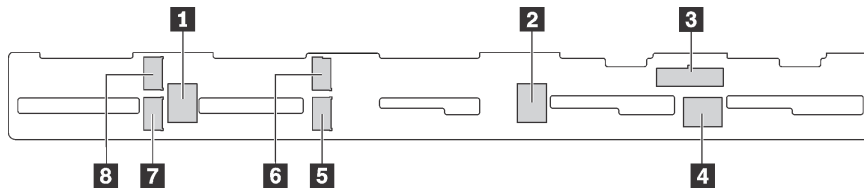
그림 30. 10개의 2.5인치 SAS/SATA/NVMe 드라이브용 백플레인의 커넥터
