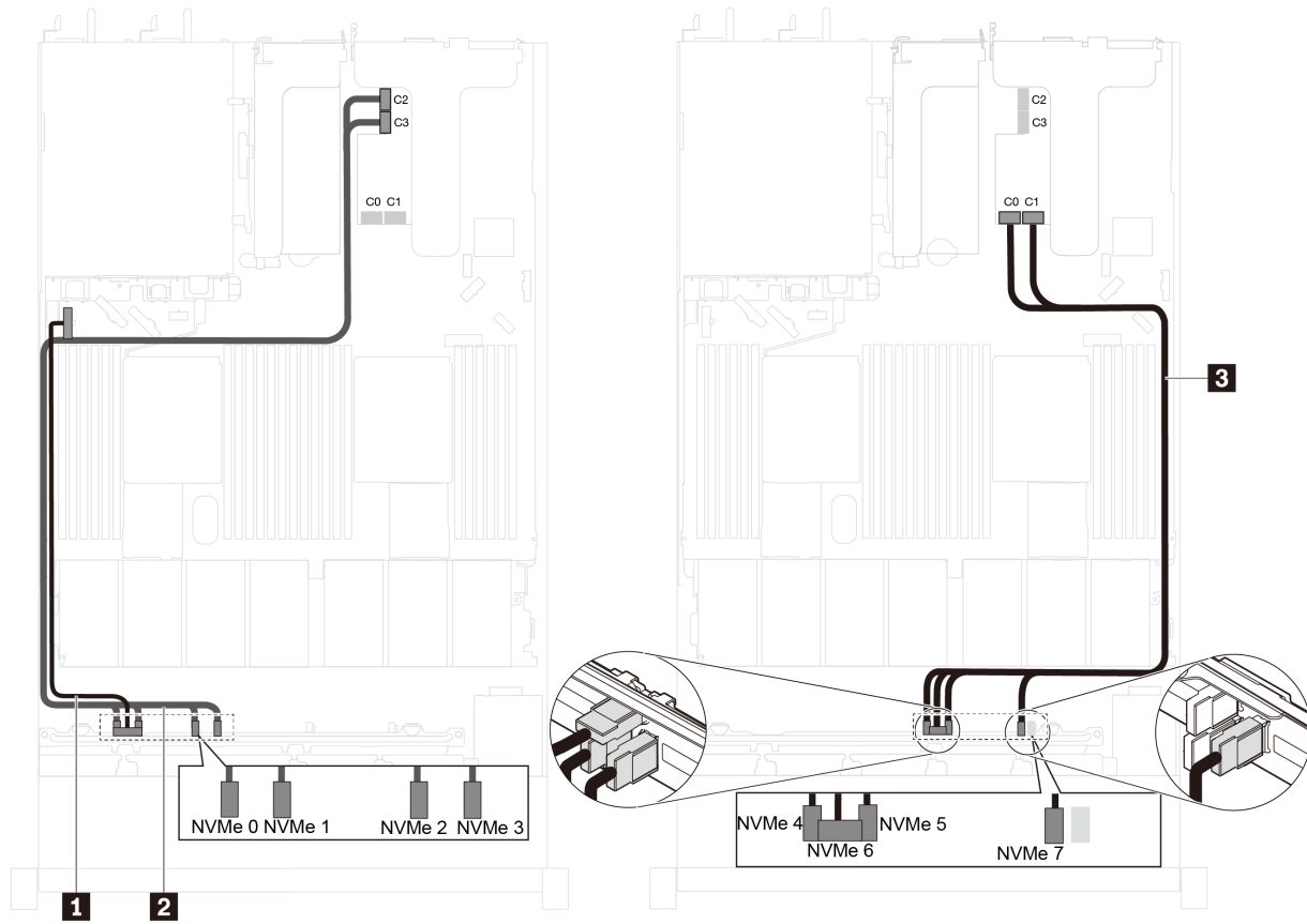
그림 44. PCIe 슬롯 2에 2.5인치 NVMe 드라이브 8개 및 1611-8P NVMe 스위치 어댑터 1개를 장착한 서버 모델의 케이블 배선
