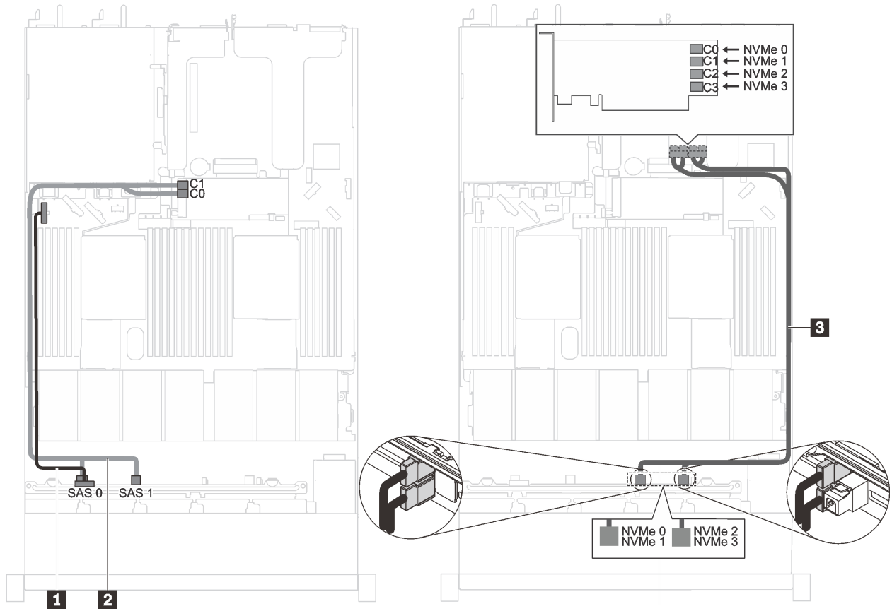
그림 34. 2.5인치 SAS/SATA 드라이브 6개, 2.5인치 NVMe 드라이브 4개, 8i HBA/RAID 어댑터 1개 및 PCIe 슬롯 2에 1610-4P NVMe 스위치 어댑터 1개가 지원되는 서버 모델의 케이블 배선
