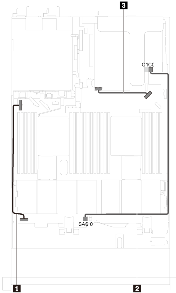
그림 21. 4개의 3.5인치 SAS/SATA 드라이브 및 1개의 전체 높이 절반 길이 GPU가 있는 서버 모델의 케이블 배선
