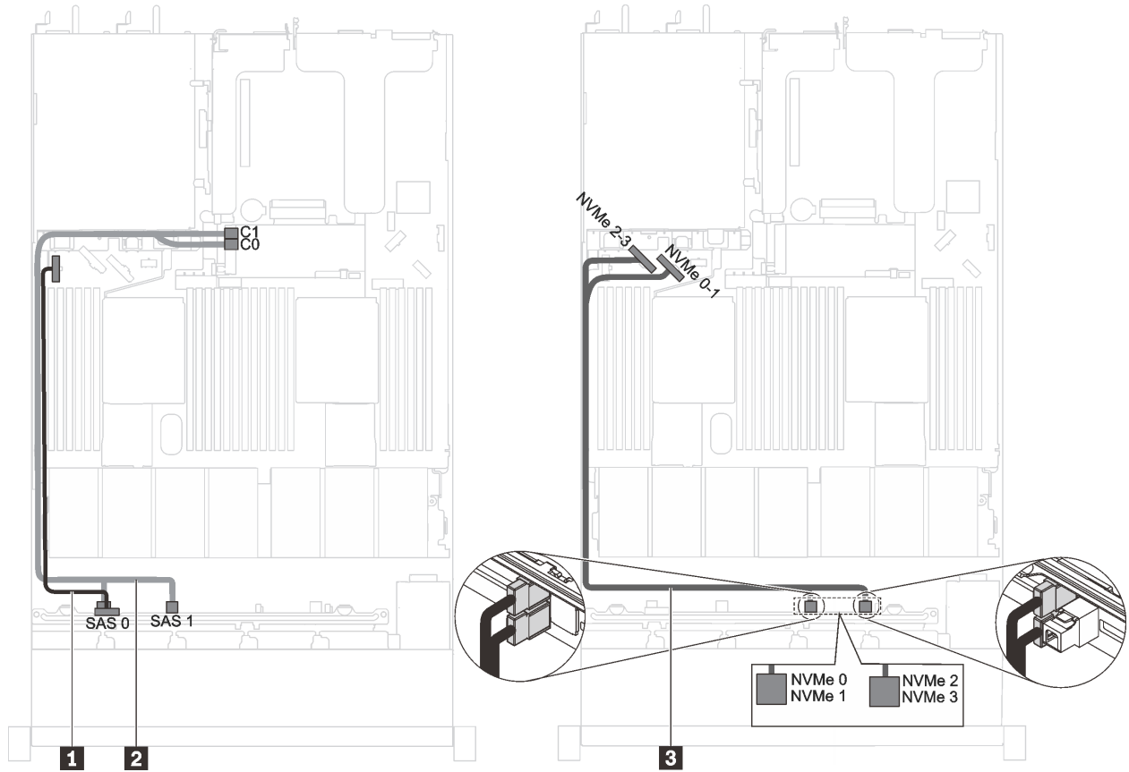
그림 32. 2.5인치 SAS/SATA 드라이브 6개, 2.5인치 NVMe 드라이브 4개, 8i HBA/RAID 어댑터 1개가 지원되는 서버 모델의 케이블 배선
