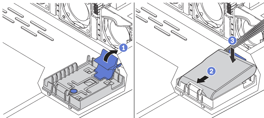
그림 86. 새시에 RAID 슈퍼 캐패시터 모듈 설치
