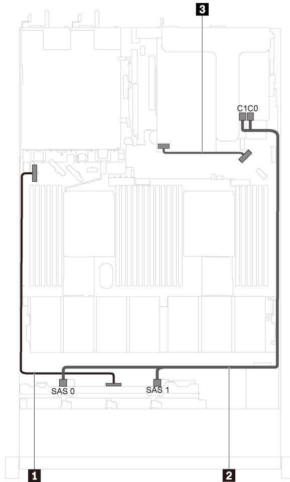
그림 29. 8개의 2.5인치 SAS/SATA 드라이브 및 1개의 전체 높이 절반 길이 GPU가 있는 서버 모델의 케이블 배선
