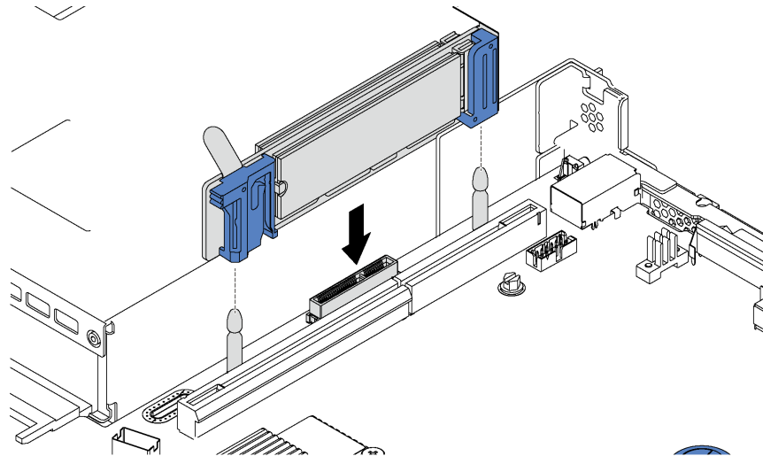
그림 66. M.2 백플레인 설치
