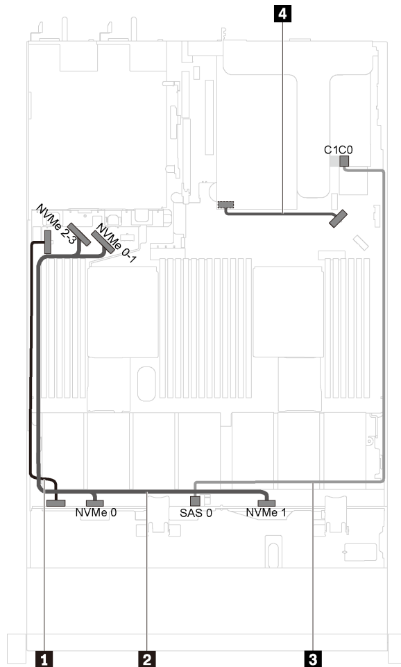
그림 24. 4개의 3.5인치 SAS/SATA/NVMe 드라이브 및 1개의 전체 높이 절반 길이 GPU가 있는 서버 모델의 케이블 배선
