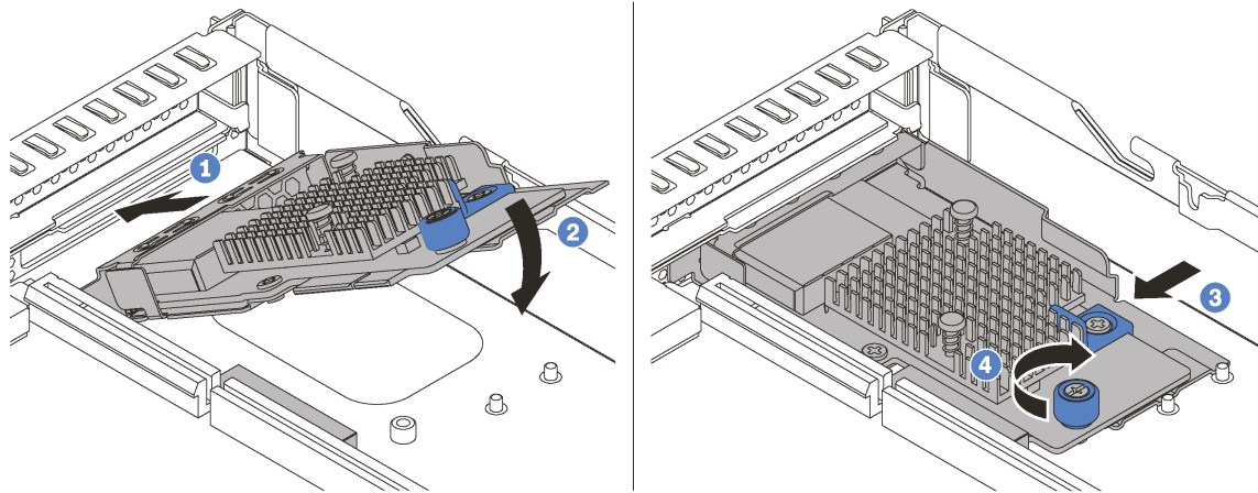
그림 68. LOM 어댑터 설치
