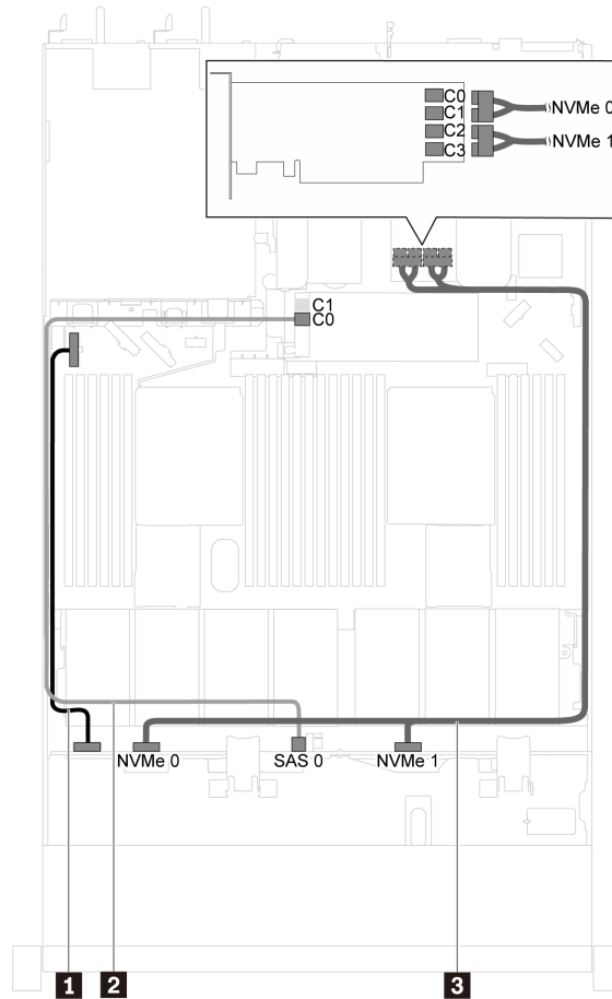
그림 25. PCIe 슬롯 2에 3.5인치 SAS/SATA/NVMe 드라이브 4개 및 1610-4P NVMe 스위치 어댑터 1개가 지원되는 서버 모델의 케이블 배선
