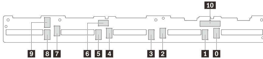
그림 38. 10개의 2.5인치 NVMe 드라이브용 백플레인의 커넥터
