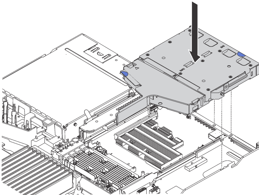
그림 62. 뒷면 핫 스왑 드라이브 어셈블리 설치
