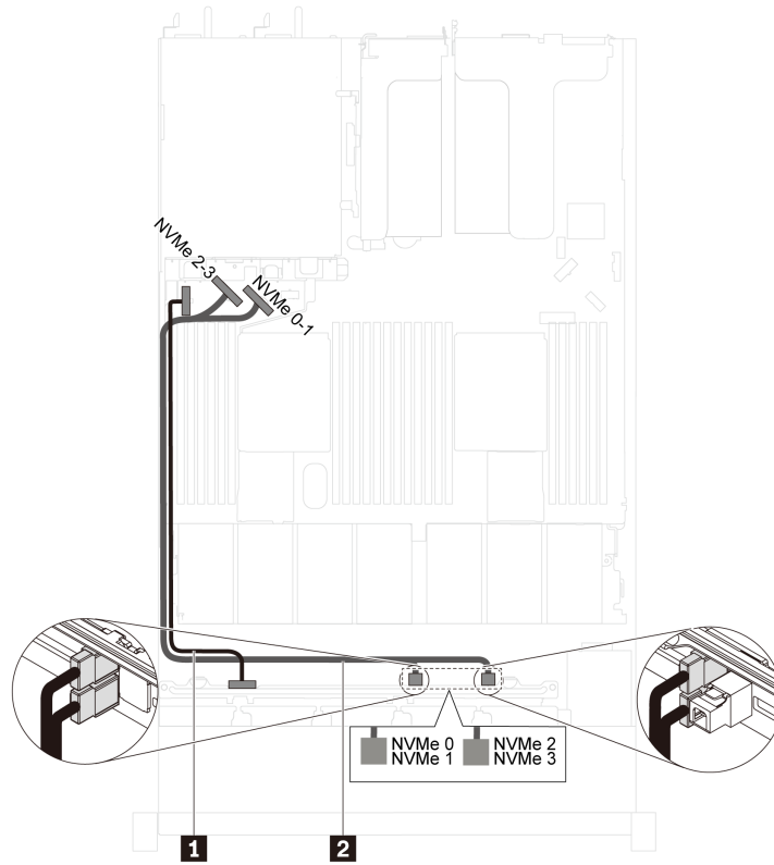
그림 37. 2.5인치 NVMe 드라이브 4개가 지원되고 RAID 어댑터가 지원되지 않는 서버 모델의 케이블 배선
