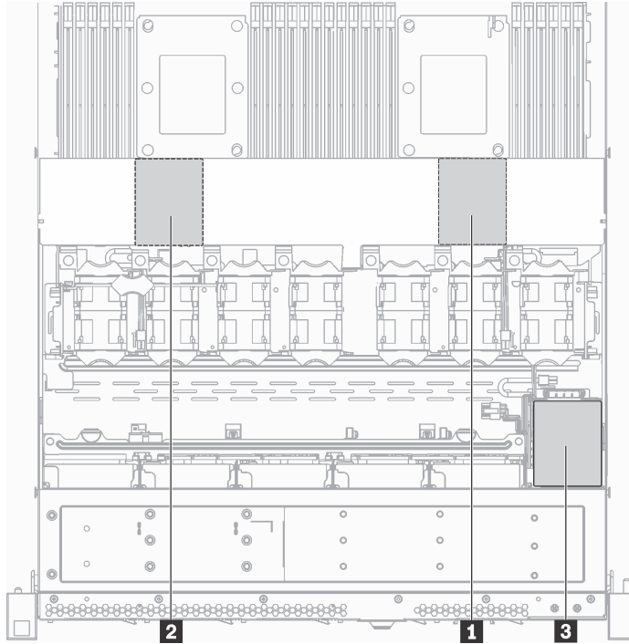
그림 83. RAID 슈퍼 캐패시터 모듈 위치
