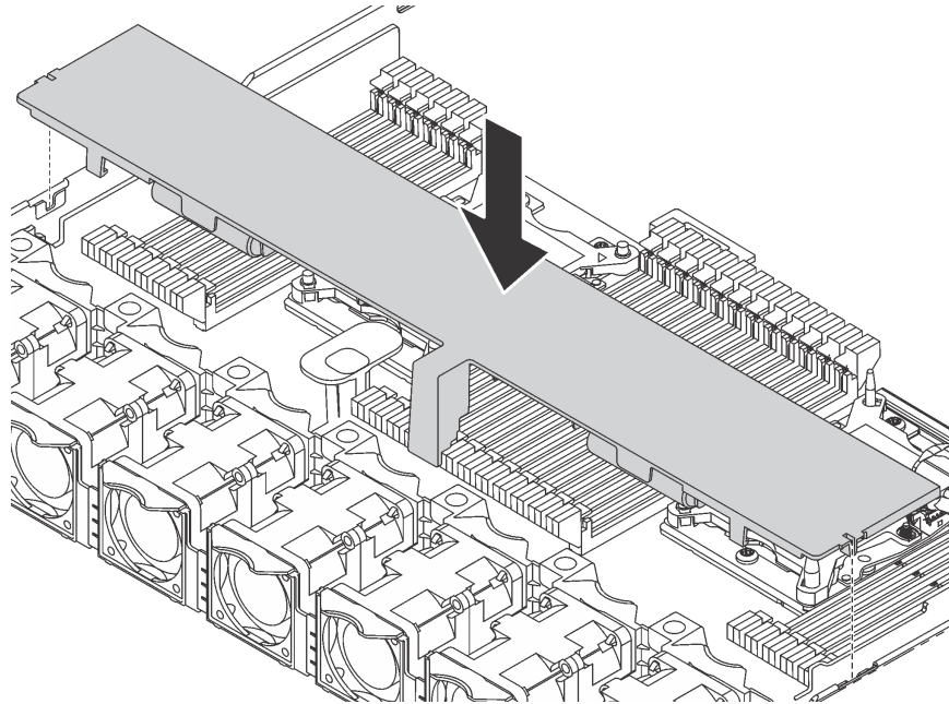
그림 87. 공기 조절 장치 설치
