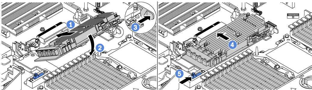
그림 58. RAID 어댑터 설치
