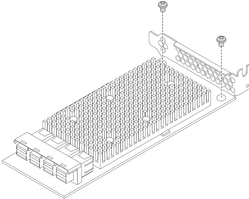
그림 77. RAID 어댑터에 로우 프로파일 브래킷 설치하기
