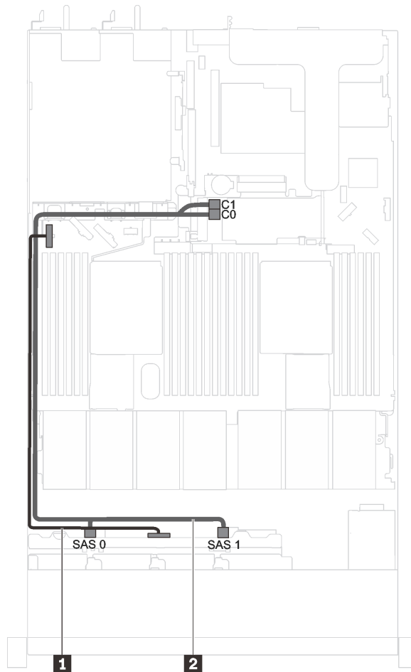
그림 27. 2.5인치 SAS/SATA 드라이브 8개 및 8i HBA/RAID 어댑터 1개가 지원되는 서버 모델의 케이블 배선
