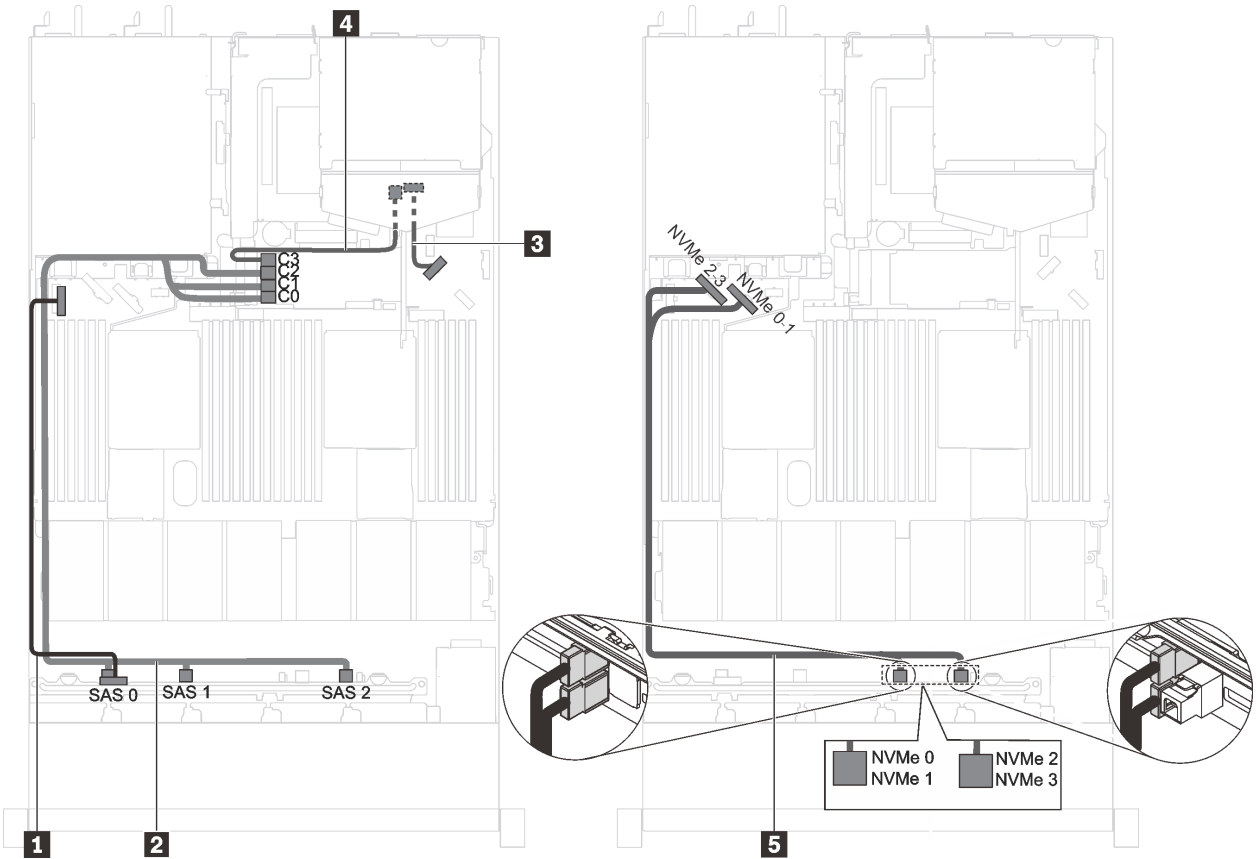
그림 31. 2.5인치 SAS/SATA 드라이브 6개, 2.5인치 SAS/SATA/NVMe 드라이브 4개, 16i HBA/RAID 어댑터 1개 및 뒷면 드라이브 어셈블리가 지원되는 서버 모델의 케이블 배선
