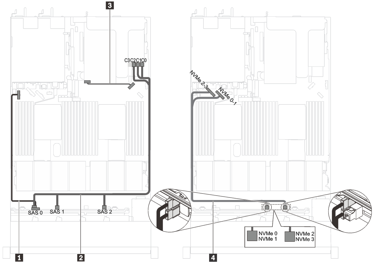
그림 33. 6개의 2.5인치 SAS/SATA 드라이브, 4개의 2.5인치 SAS/SATA/NVMe 드라이브 및 1개의 전체 높이 절반 길이 GPU가 있는 서버 모델의 케이블 배선
