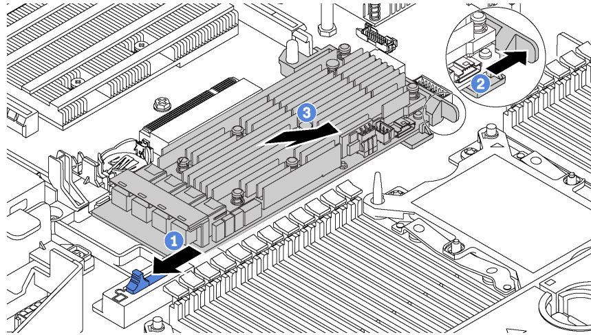
그림 76. RAID 어댑터 제거
