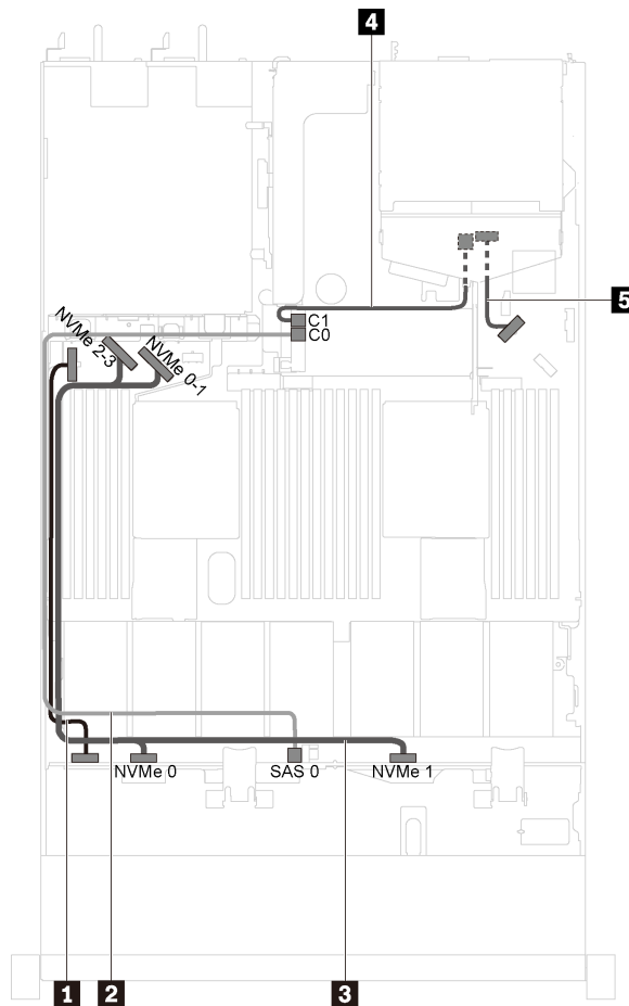
그림 23. 4개의 3.5인치 SAS/SATA/NVMe 드라이브 및 뒷면 드라이브 어셈블리가 있는 서버 모델의 케이블 배선
