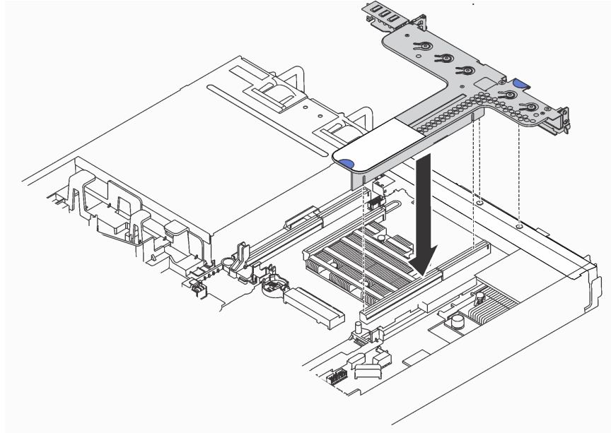
그림 75. 라이저 어셈블리 설치
