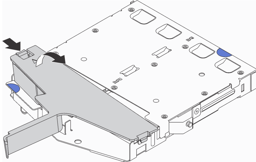
그림 59. 공기 조절 장치 제거
