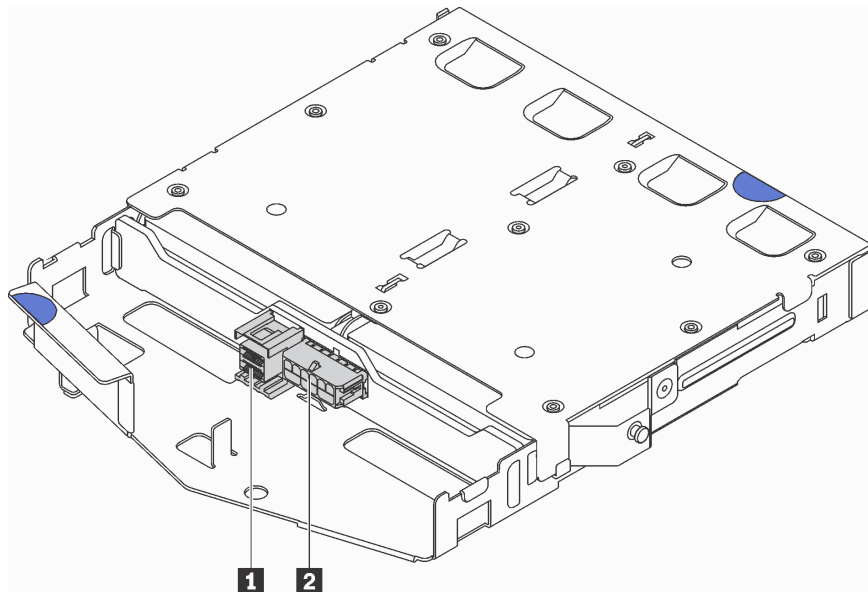
그림 60. 뒷면 백플레인 커넥터
