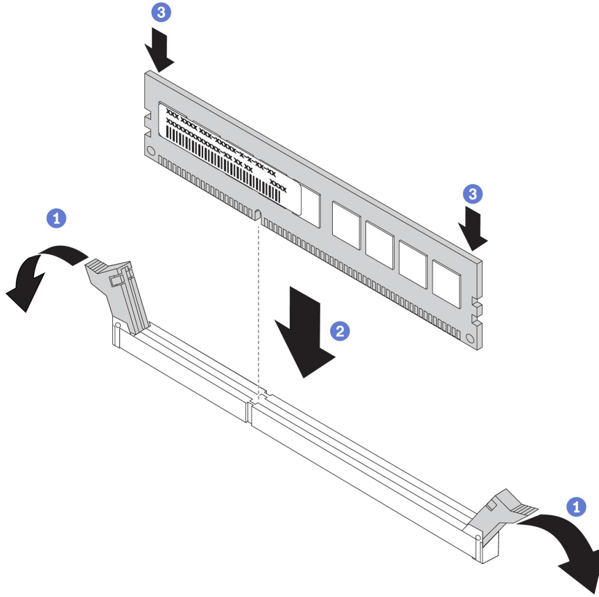
그림 52. 메모리 모듈 설치
