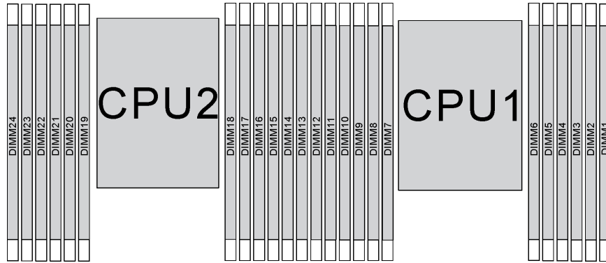
그림 53. 시스템 보드의 메모리 모듈 슬롯
