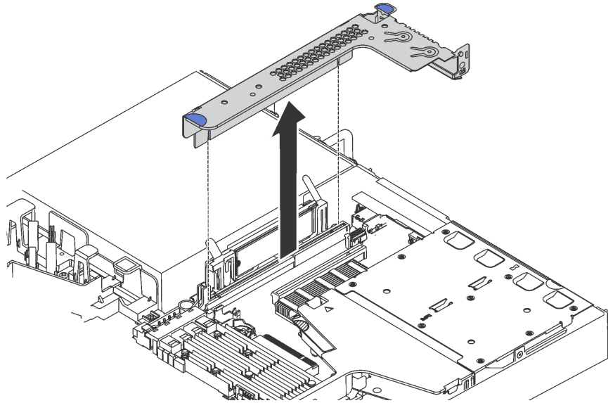
그림 78. 라이저 어셈블리 제거
