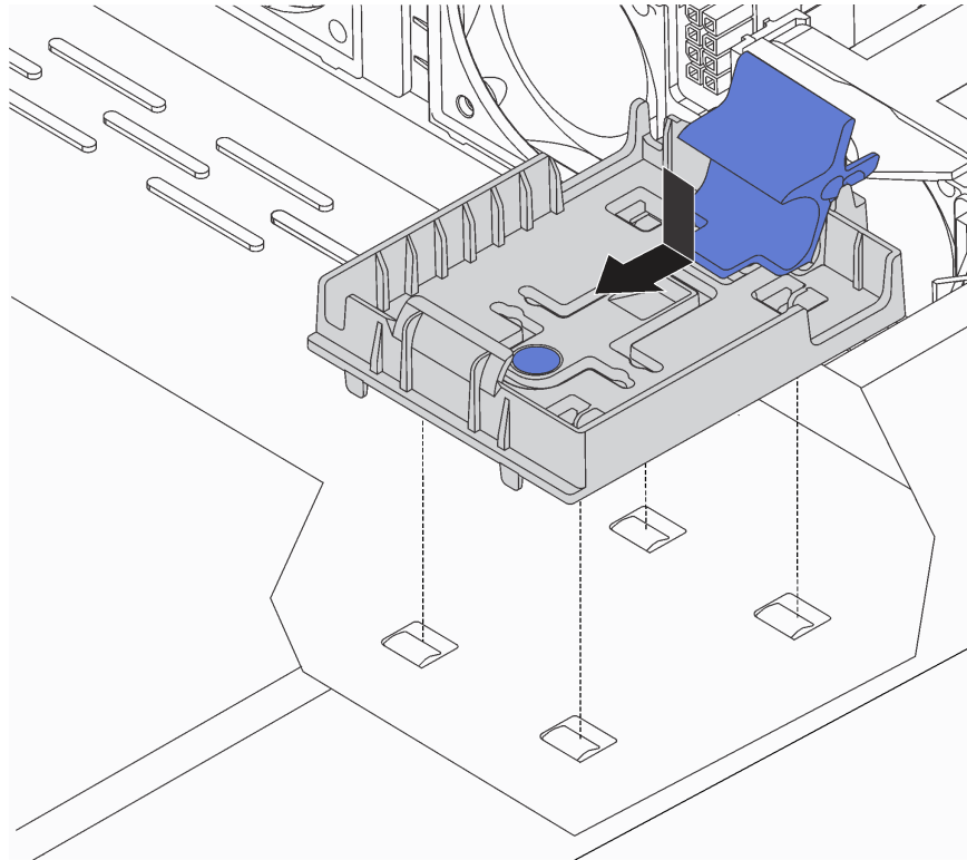
그림 85. RAID 슈퍼 캐패시터 모듈 홀더 설치
