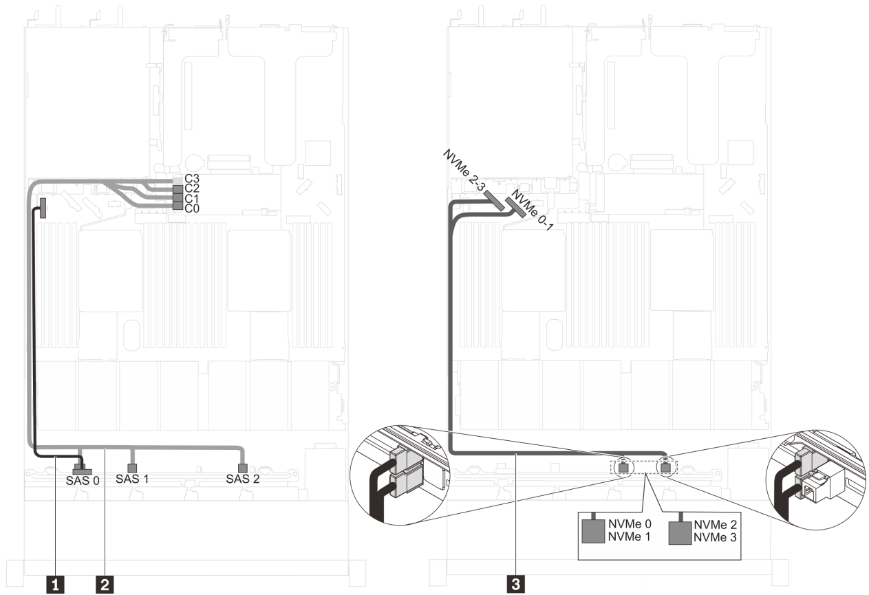
图 35. 配备 Intel Xeon 6154/6254/6240Y 处理器、四个 2.5 英寸 SAS/SATA/NVMe 硬盘和一个 16i HBA/RAID 适配器的服务器型号的线缆布放
