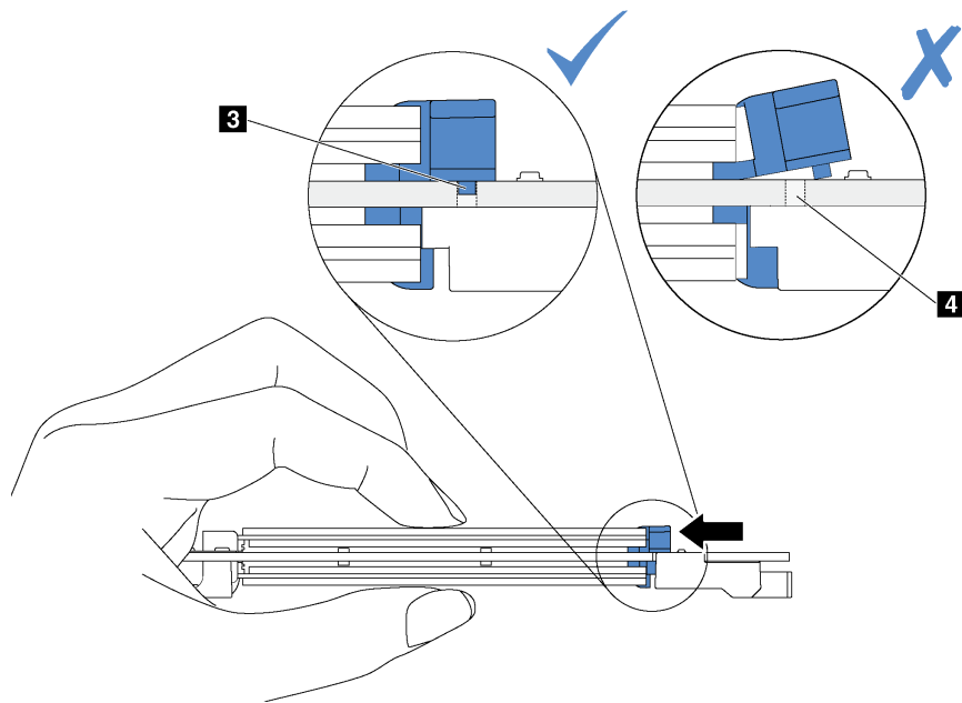
图 65. 关于滑动固定器的说明
