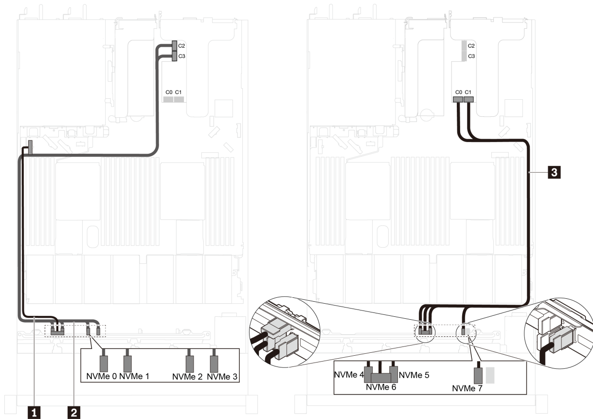
图 44. 配备八个 2.5 英寸 NVMe 硬盘并在 PCIe 插槽 2 中装有一个 NVMe 1611-8P 交换适配器的服务器型号的线缆布放
