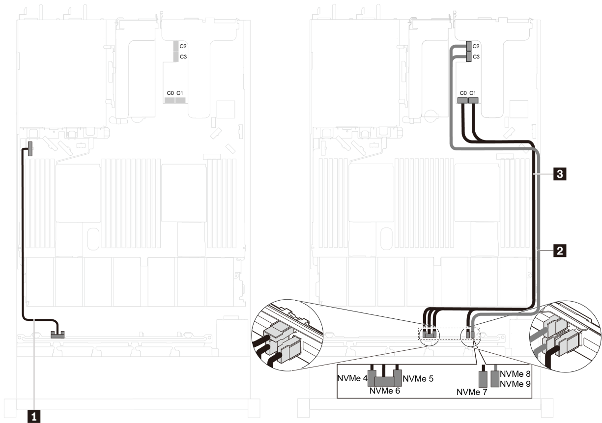
图 41. 配备十个 2.5 英寸 NVMe 硬盘并在 PCIe 插槽 2 中装有一个 NVMe 1611-8P 交换适配器的服务器型号的线缆布放
