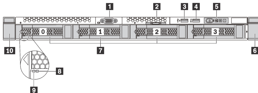
图 7. 配备四个 3.5 英寸硬盘插槽的服务器型号的前视图
