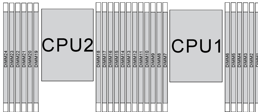
图 54. 主板上的内存条插槽
