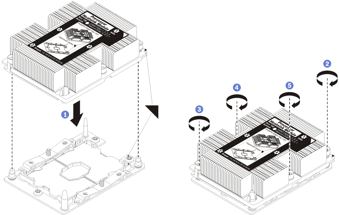
图 50. 安装 PHM
