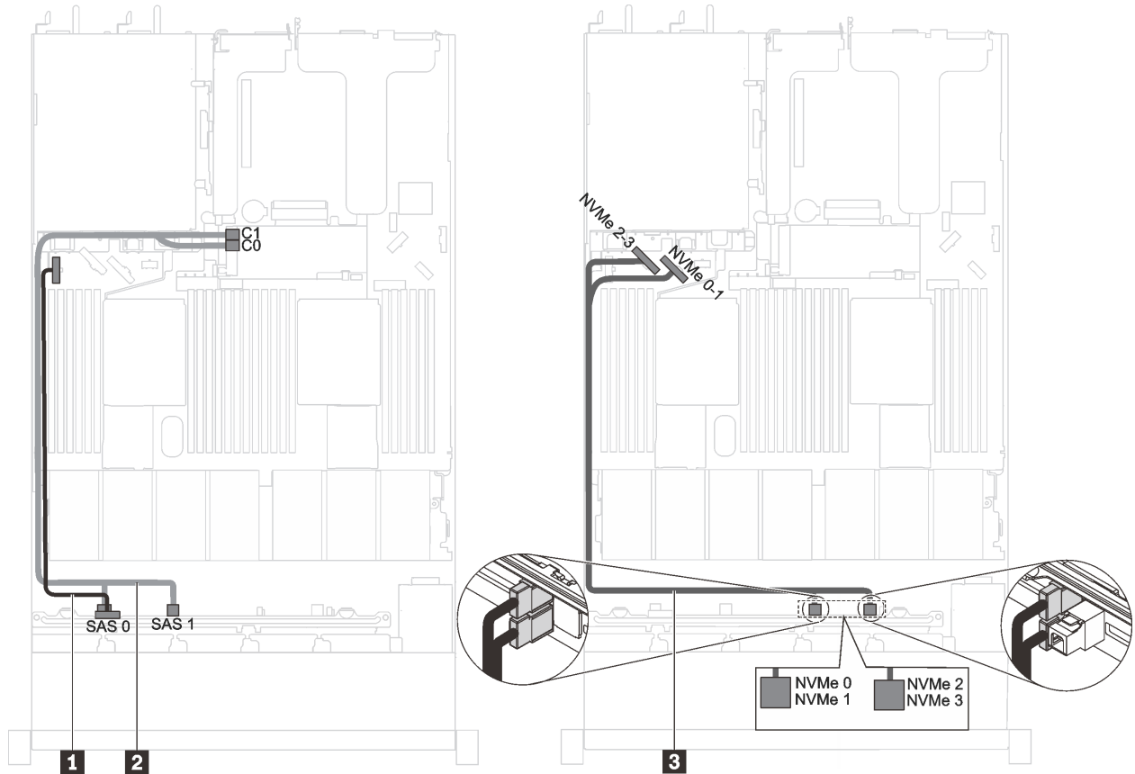
图 32. 配备六个 2.5 英寸 SAS/SATA 硬盘、四个 2.5 英寸 NVMe 硬盘和一个 8i HBA/RAID 适配器的服务器型号的线缆布放
