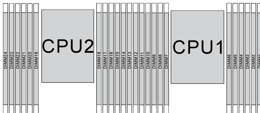
图 53. 主板上的内存条插槽
