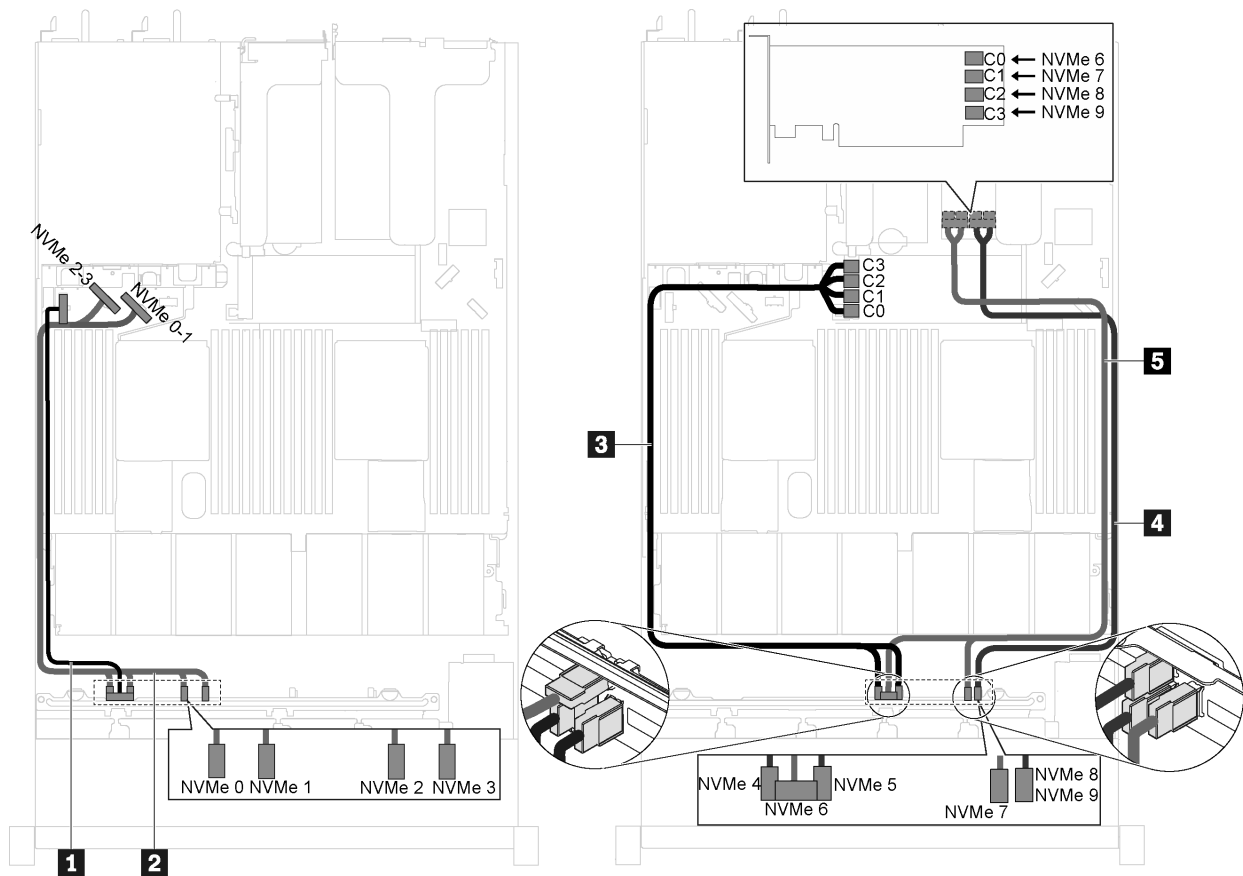
图 40. 装有十个 2.5 英寸 NVMe 硬盘、在 PCIe 插槽 2 中装有一个 1610-4P NVMe 交换适配器并在 RAID 适配器插槽中装有一个 810-4P NVMe 交换适配器的服务器型号的线缆布放
