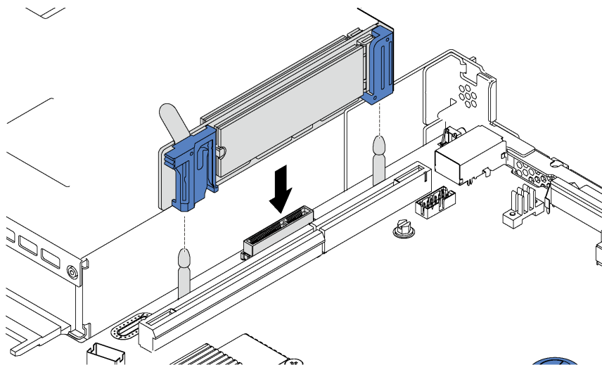
图 66. 安装 M.2 背板
