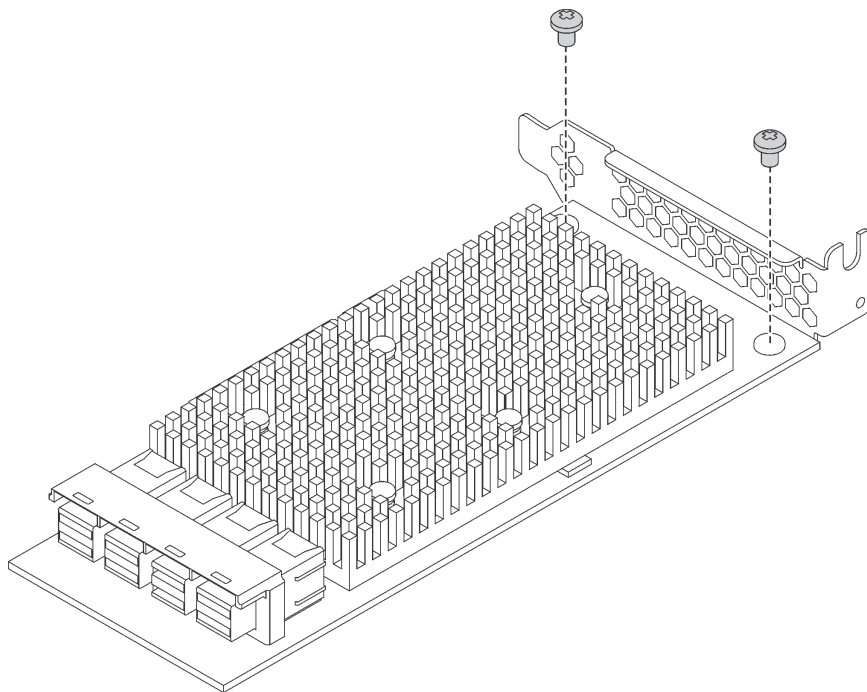
图 77. 将半高型支架安装到 RAID 适配器上
