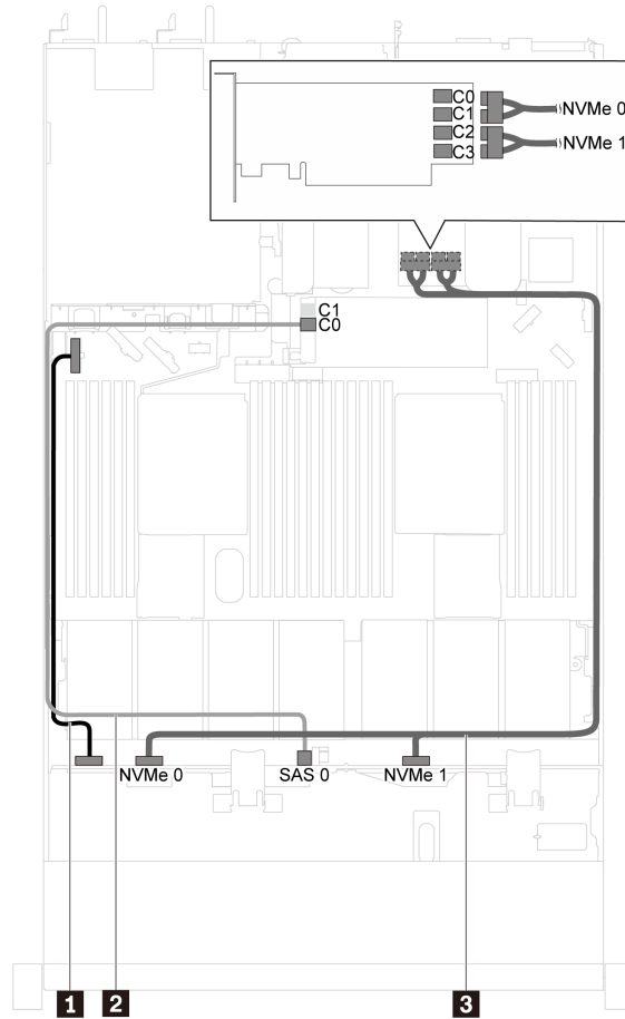
图 25. 配备四个 3.5 英寸 SAS/SATA/NVMe 硬盘和一个 1610-4P NVMe 交换适配器 (PCIe 插槽 2 中) 的服务器型号的线缆布放
