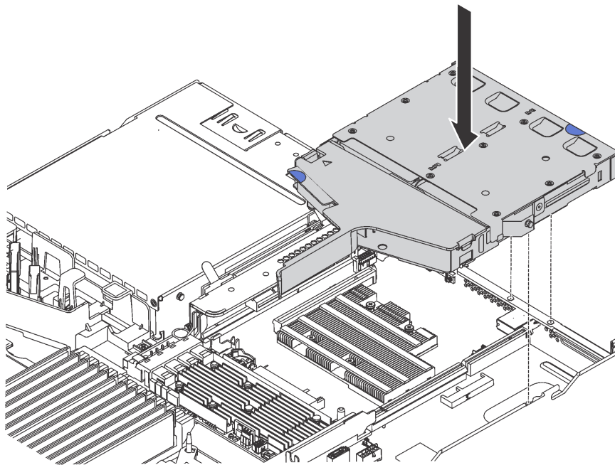
图 62. 安装背面热插拔硬盘组合件
