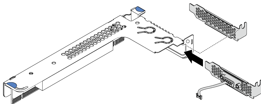
图 79. 安装串口模块
