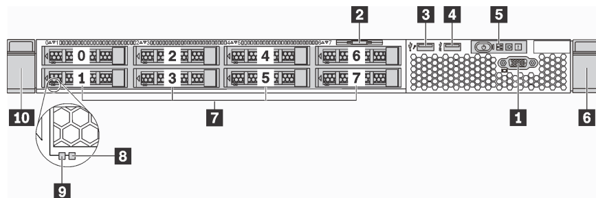
图 8. 配备八个 2.5 英寸硬盘插槽的服务器型号的前视图
