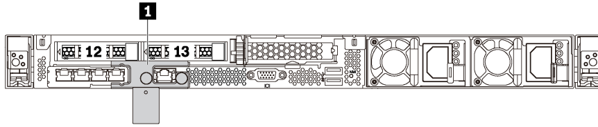
图 14. 配备装运支架的服务器型号的后视图
