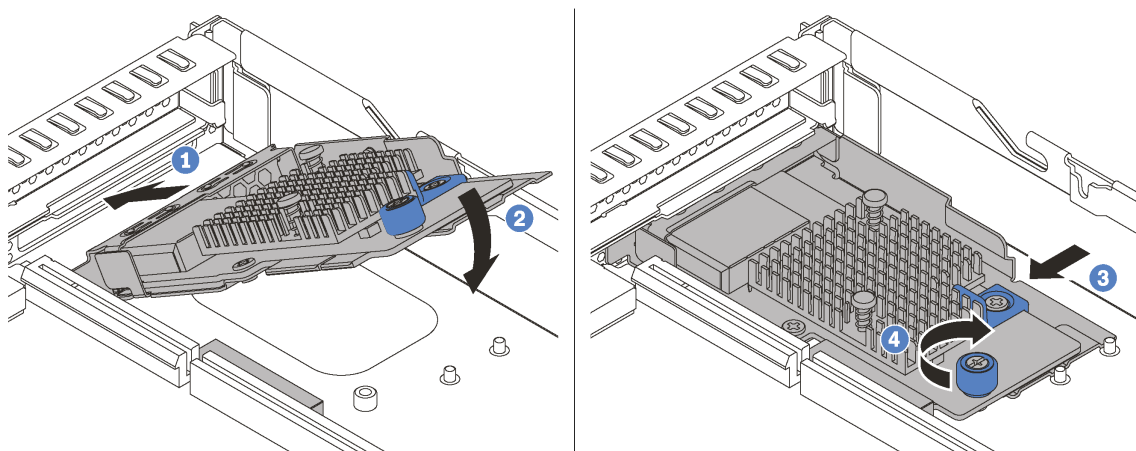
图 68. 安装 LOM 适配器
