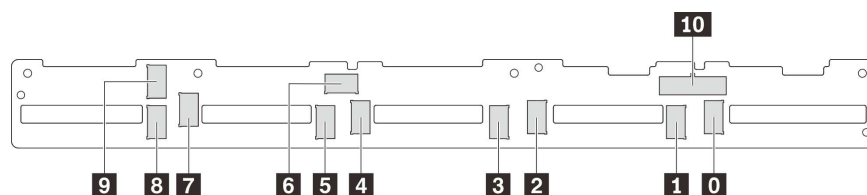
图 38. 用于十个 2.5 英寸 NVMe 硬盘的背板上的接口
