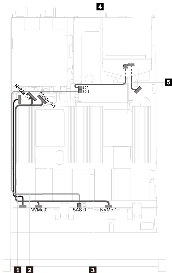
图 23. 装有四个 3.5 英寸 SAS/SATA/NVMe 硬盘和背面硬盘组合件的服务器型号的线缆布放
