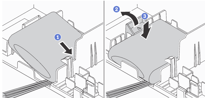
图 82. 在导风罩底部安装 RAID 超级电容器模块
