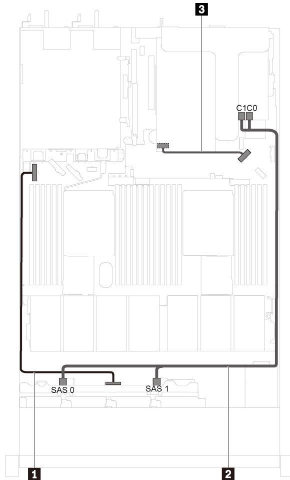
图 29. 装有八个 2.5 英寸 SAS/SATA 硬盘和全高半长型 GPU 的服务器型号的线缆布放
