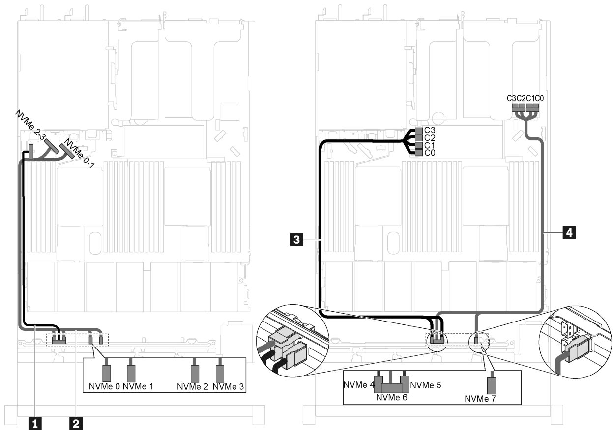
图 43. 装有八个 2.5 英寸 NVMe 硬盘、在 PCIe 插槽 1 中装有一个 810-4P NVMe 交换适配器并在 RAID 适配器插槽中装有一个 810-4P NVMe 交换适配器的服务器型号的线缆布放
