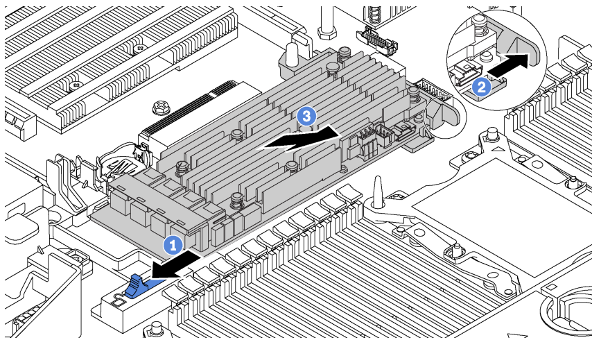
图 76. 卸下 RAID 适配器
