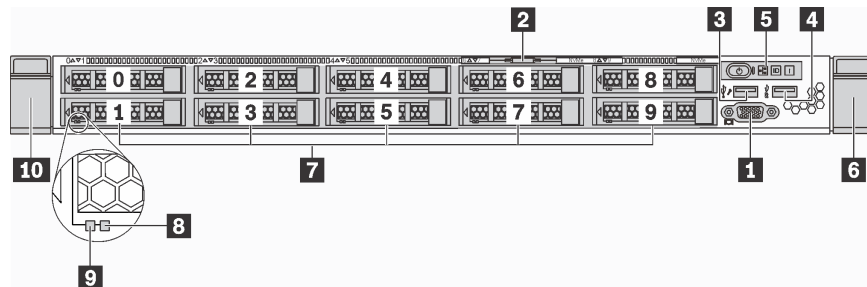
图 9. 配备十个 2.5 英寸硬盘插槽的服务器型号的前视图
