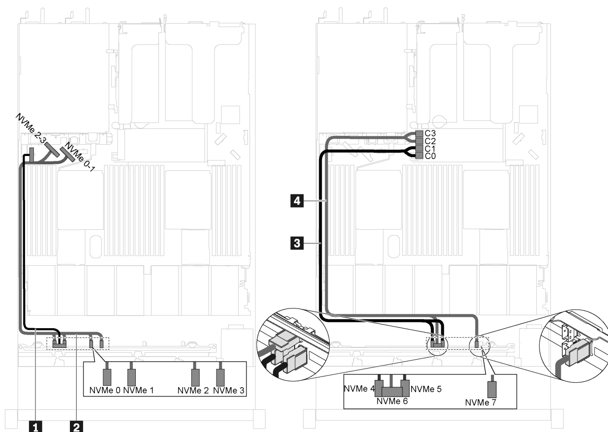
图 42. 装有八个 2.5 英寸 NVMe 硬盘并在 RAID 适配器插槽中装有一个 810 4 P NVMe 交换适配器的服务器型号的线缆布放
