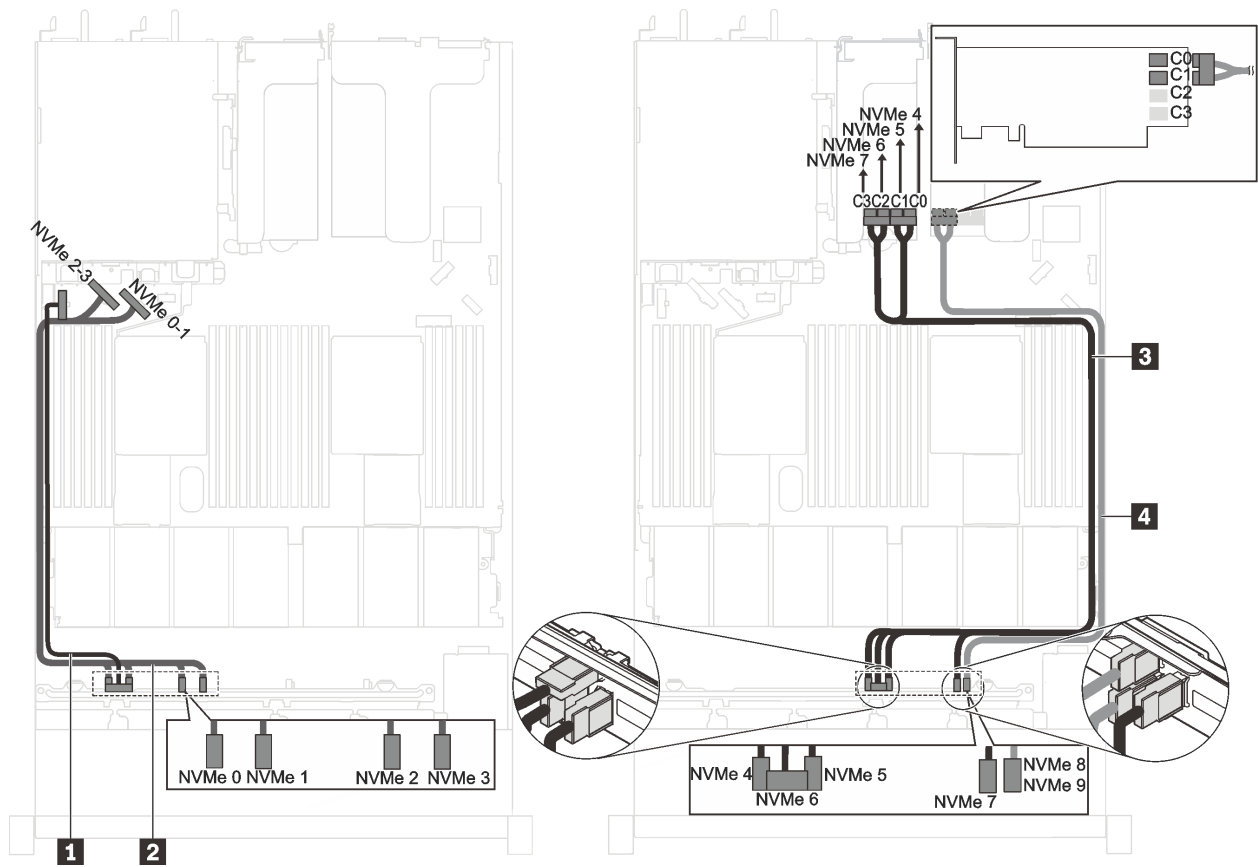
图 39. 装有十个 2.5 英寸 NVMe 硬盘、在 PCIe 插槽 2 中装有一个 1610-4P NVMe 交换适配器并在 PCIe 插槽 3 中装有一个 1610-4P NVMe 交换适配器的服务器型号的线缆布放
