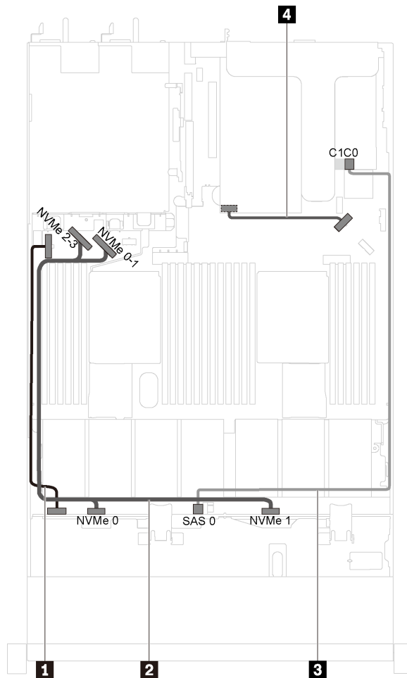
图 24. 装有四个 3.5 英寸 SAS /SATA/NVMe 硬盘和全高半长型 GPU 的服务器型号的线缆布放
