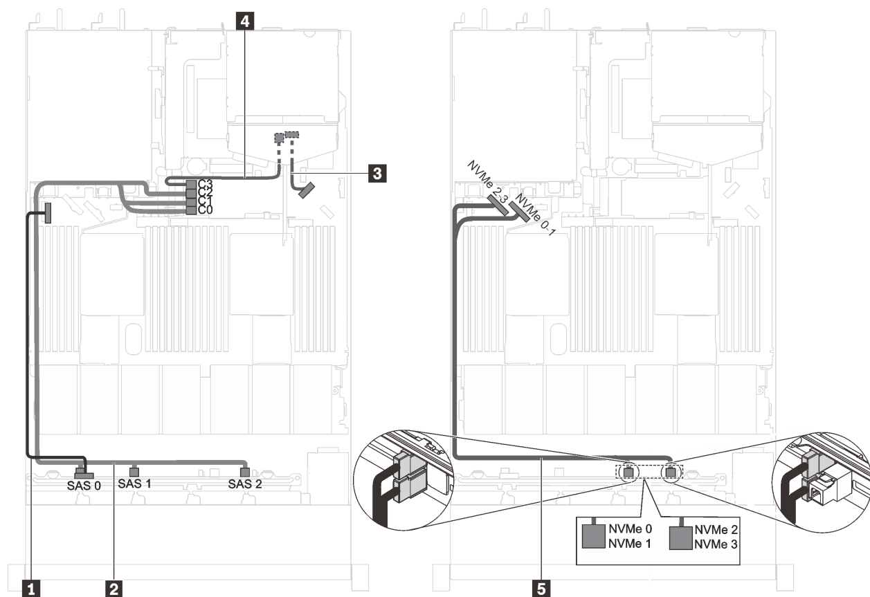
图 31. 配备六个 2.5 英寸 SAS/SATA 硬盘、四个 2.5 英寸 SAS/SATA/NVMe 硬盘、一个 16i HBA/RAID 适配器和背面硬盘组合件的服务器型号的线缆布放
