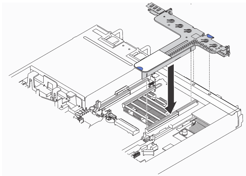
图 75. 安装转接卡组合件
