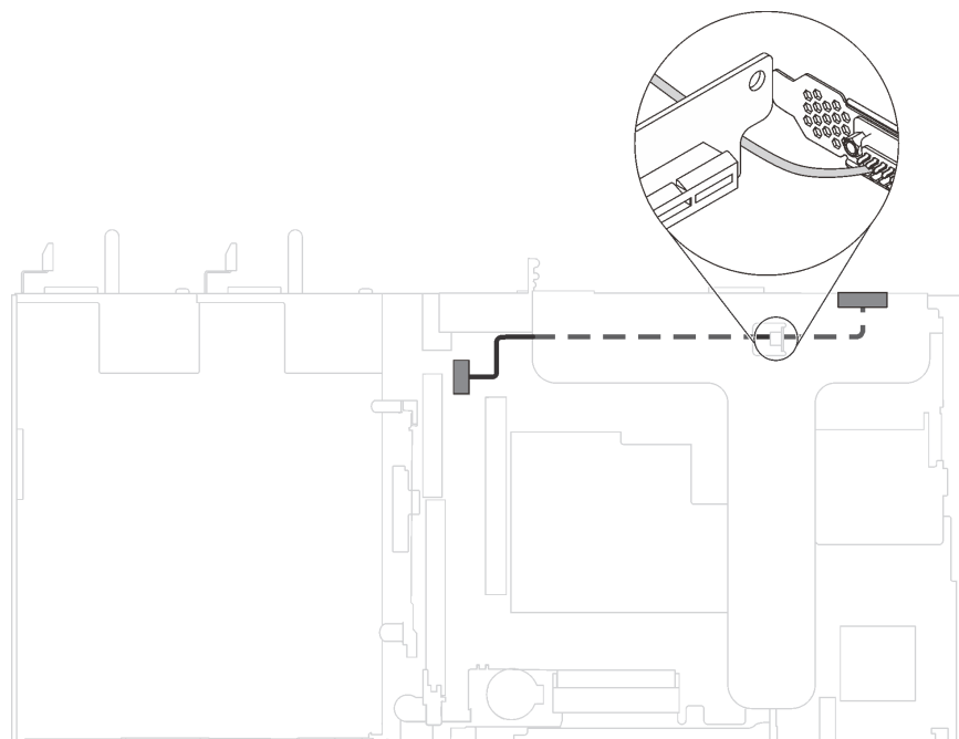
图 80. 安装在 PCIe 插槽 1 中的串口模块的线缆布放
