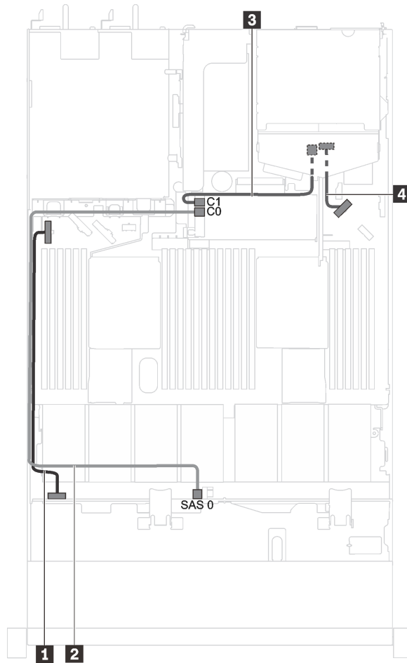
图 20. 配备四个 3.5 英寸 SAS/SATA 硬盘和背面硬盘组合件的服务器型号的线缆布放
