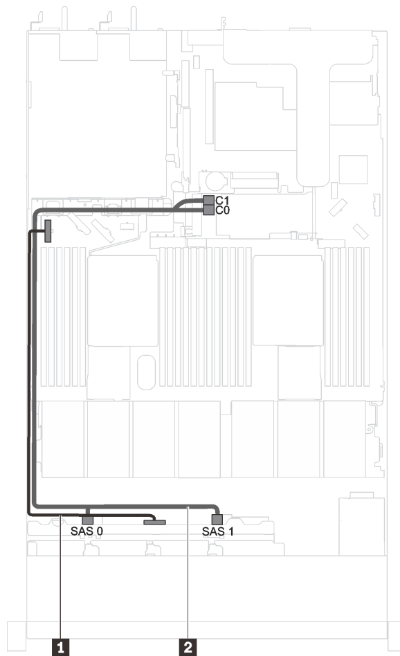
图 27. 配备八个 2.5 英寸 SAS/SATA 硬盘和一个 8i HBA/RAID 适配器的服务器型号的线缆布放
