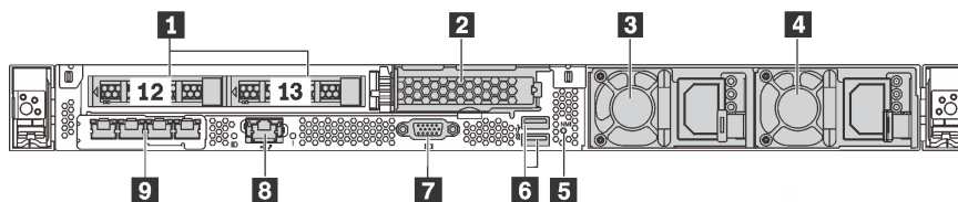
图 13. 配备两个热插拔硬盘插槽和一个 PCIe 插槽的服务器型号的后视图
