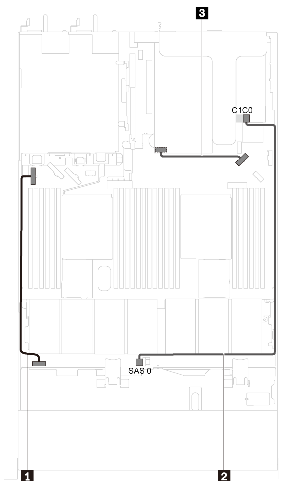
图 21. 装有四个 3.5 英寸 SAS/SATA 硬盘和全高半长型 GPU 的服务器型号的线缆布放
