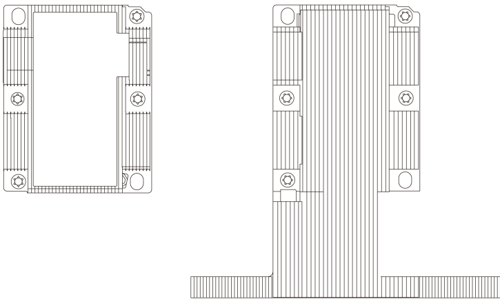
图 5. 两种类型的散热器
