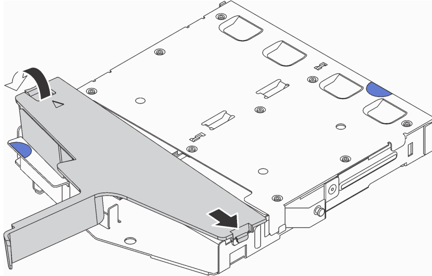
图 61. 安装导风罩
