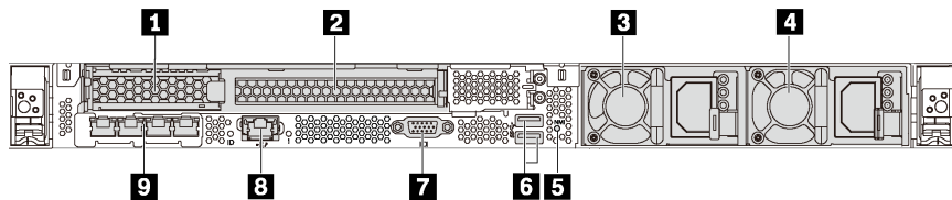
图 12. 配备两个 PCIe 插槽的服务器型号的后视图
