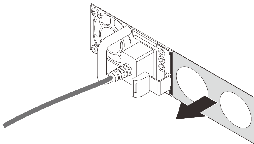
图 56. 卸下热插拔电源模块填充件
