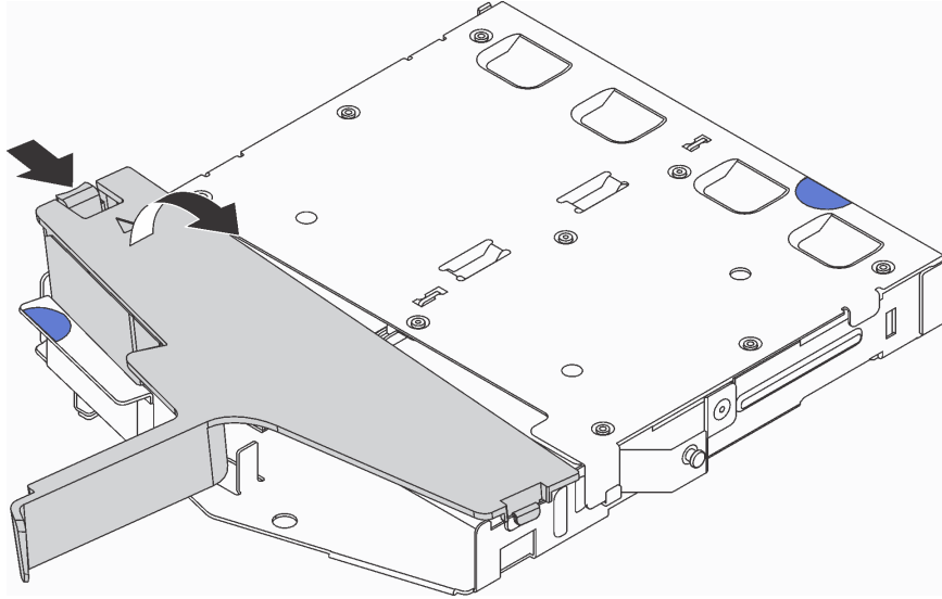
图 59. 卸下导风罩
