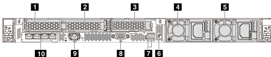
图 11. 配备三个 PCIe 插槽的服务器型号的后视图
