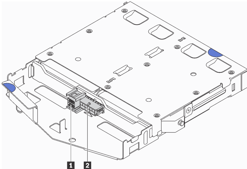
图 60. 背面背板接口
