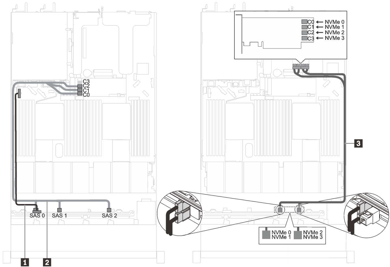
图 36. 配备六个 2.5 英寸 SAS/SATA 硬盘、四个 2.5 英寸 NVMe 硬盘、一个 16i HBA/RAID 适配器和一个 1610-4P NVMe 交换适配器（装入 PCIe 插槽 2 中）的服务器型号的线缆布放
