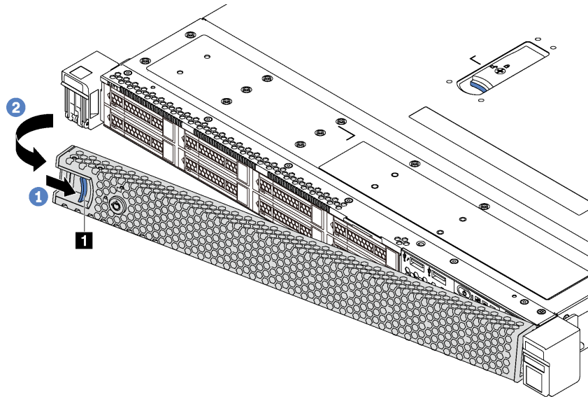
图 47. 卸下安全挡板
