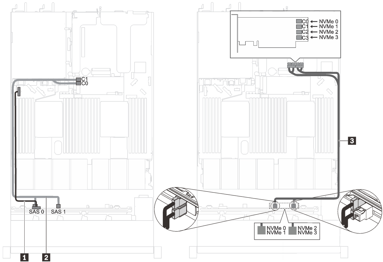
图 34. 配备六个 2.5 英寸 SAS/SATA 硬盘、四个 2.5 英寸 NVMe 硬盘、一个 8i HBA/RAID 适配器和一个 1610-4P NVMe 交换适配器（装入 PCIe 插槽 2 中）的服务器型号的线缆布放
