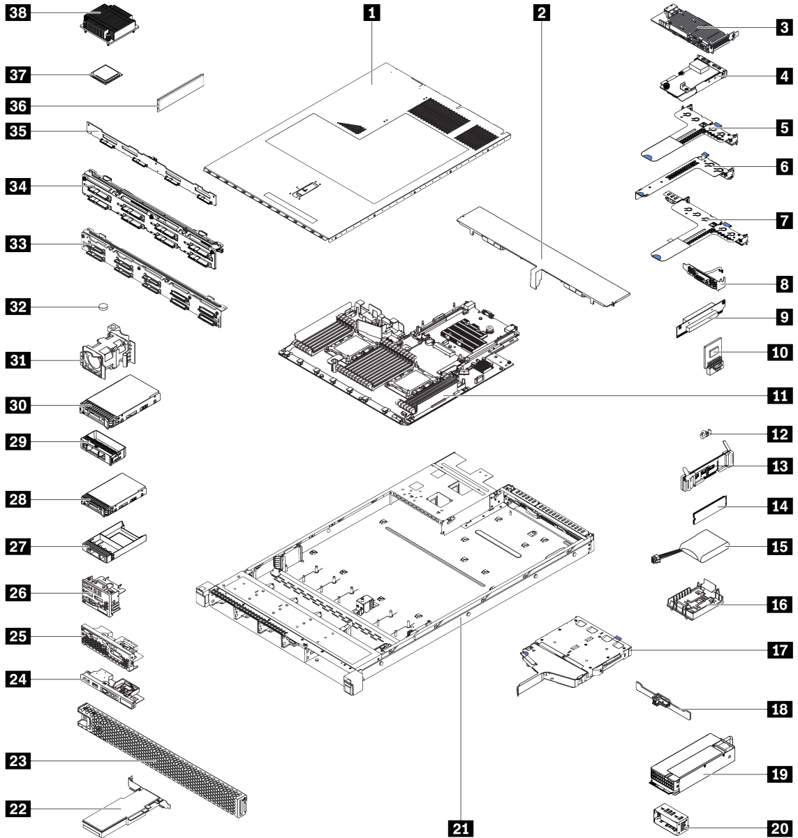
图 45. 服务器组件
