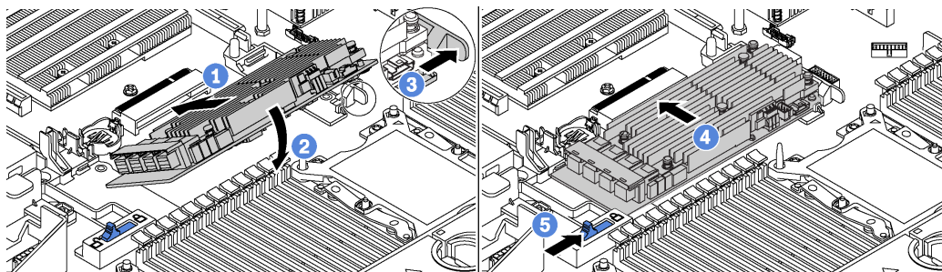
图 58. 安装 RAID 适配器
