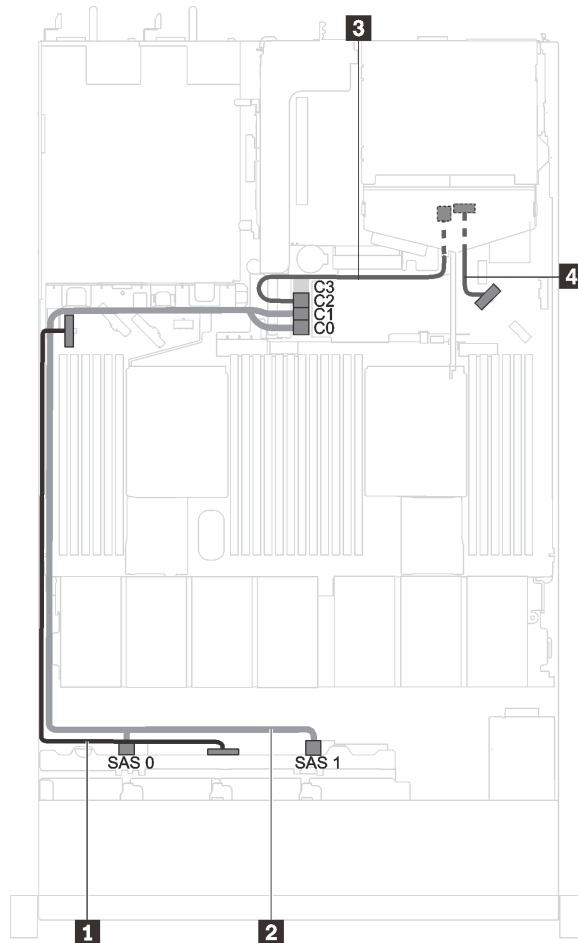
图 28. 配备八个 2.5 英寸 SAS/SATA 硬盘、一个 16i HBA/RAID 适配器和背面硬盘组合件的服务器型号的线缆布放
