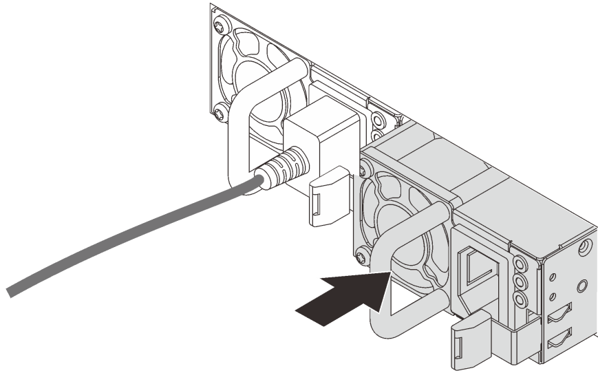
图 57. 安装热插拔电源模块
