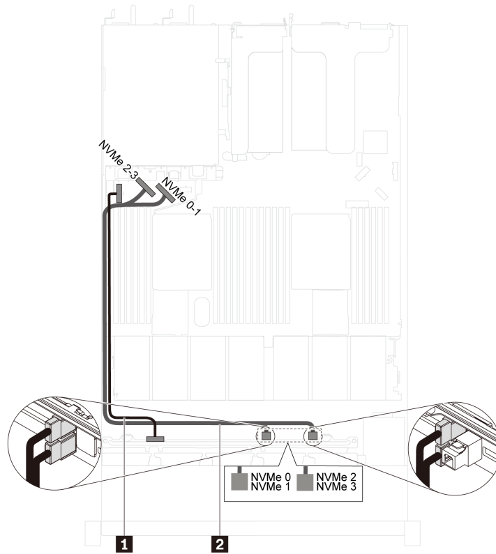
图 37. 配备四个 2.5 英寸 NVMe 硬盘且无 RAID 适配器的服务器型号的线缆布放
