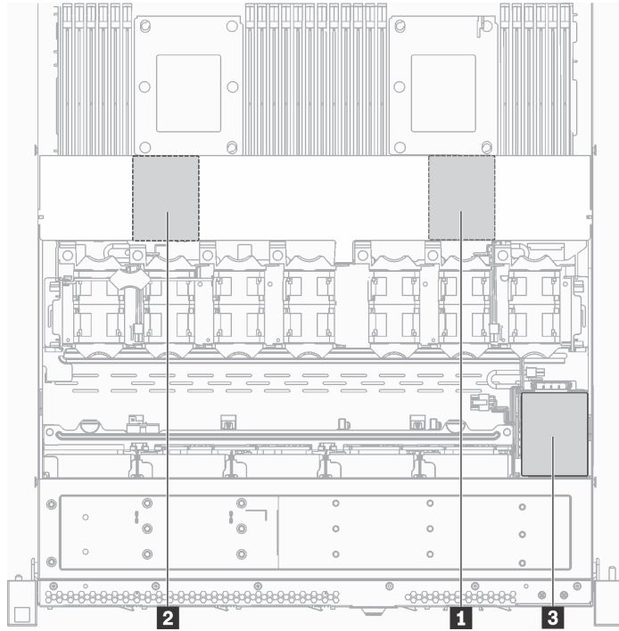
图 83. RAID 超级电容器模块位置
