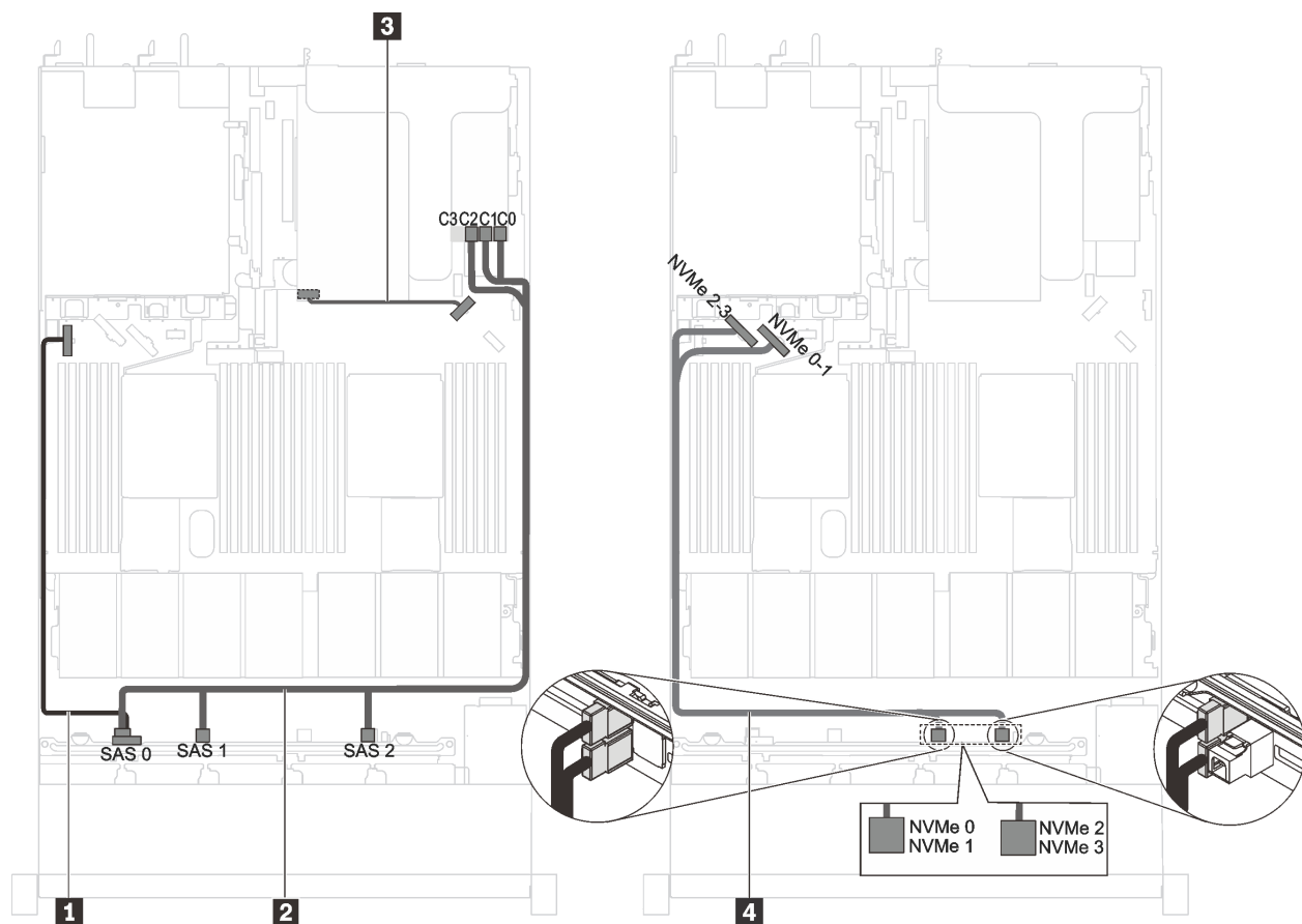
图 33. 装有六个 2.5 英寸 SAS/SATA 硬盘、四个 2.5 英寸 SAS /SATA/NVMe 硬盘和全高半长型 GPU 的服务器型号的线缆布放
