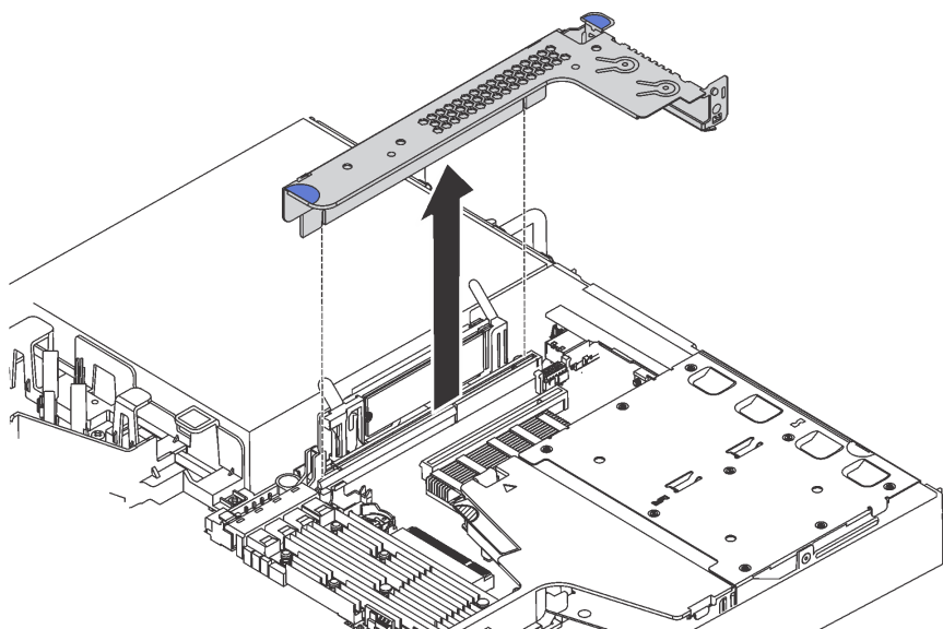
图 78. 卸下转接卡组合件
