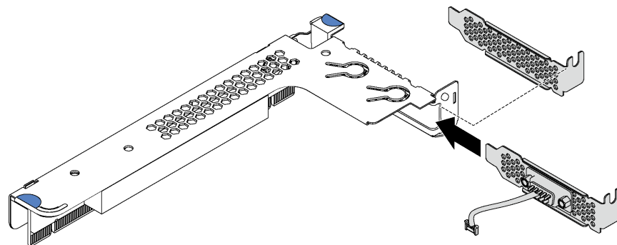
圖例 79. 序列埠模組安裝
