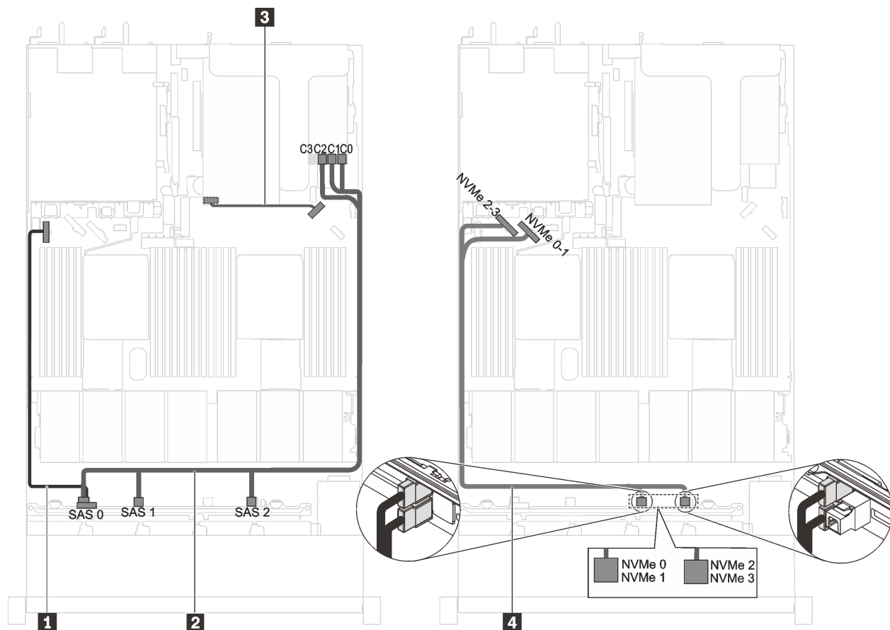
圖例 33. 配備六個 2.5 吋 SAS/SATA 硬碟、四個 2.5 吋 SAS/SATA/NVMe 硬碟和全高半長 GPU 之伺服器型號的纜線佈線
