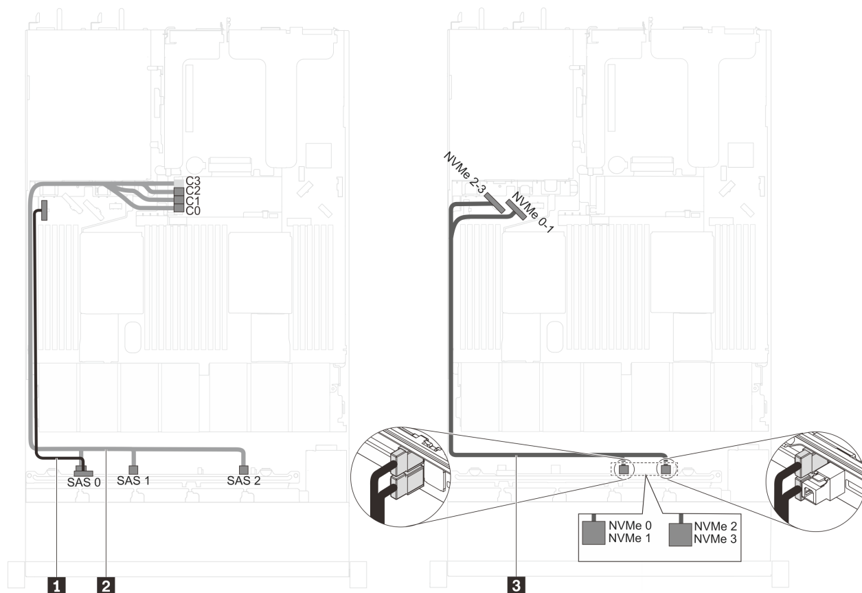
圖例 35. 配備 Intel Xeon 6154、6254 和 6240Y 處理器、四部 2.5 吋 SAS/SATA/NVMe 硬碟和一個 16i HBA/RAID 配接卡之伺服器型號的纜線佈線
