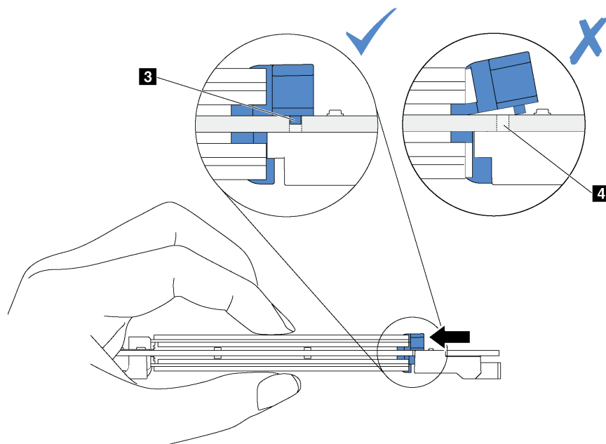
圖例 65. 滑動固定器指示
