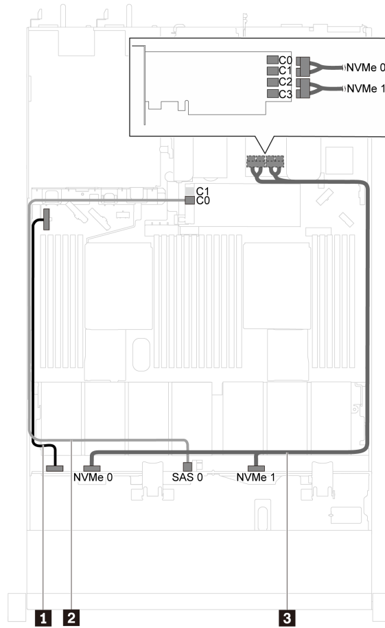
圖例 25. 配備四個 3.5 吋 SAS/SATA/NVMe 硬碟及一個 1610-4P NVMe 交換器配接卡 ( 在 PCIe 插槽 2 中 ) 之伺服器型號的纜線佈線
