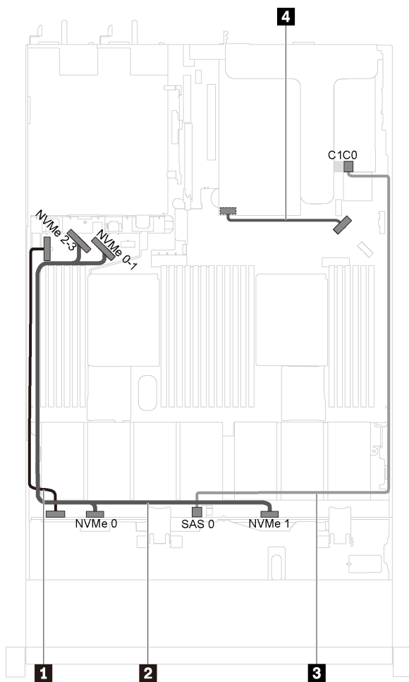
圖例 24. 配備四個 3.5 吋 SAS/SATA/NVMe 硬碟和全高半長 GPU 之伺服器型號的纜線佈線
