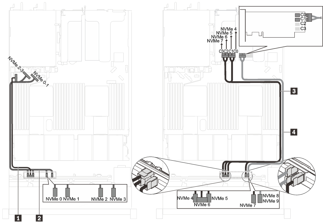
圖例 39. 配備十個 2.5 吋 NVMe 硬碟、一個 1610-4P NVMe 交換器配接卡 ( 在 PCIe 插槽 2 中 ) 以及一個 1610-4P NVMe 交換器配接卡 ( 在 PCIe 插槽 3 中 ) 之伺服器型號的纜線佈線
