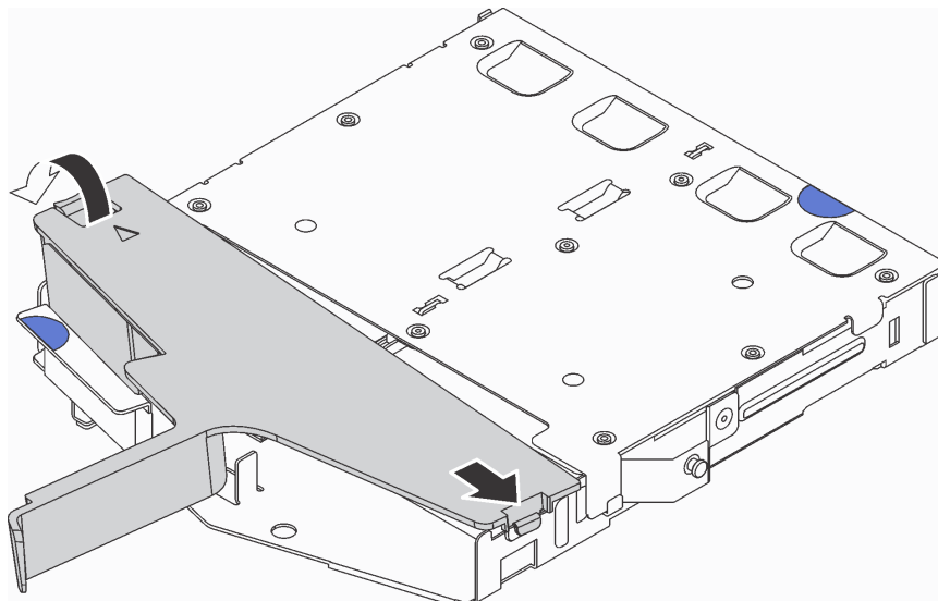
圖例 61. 安裝空氣擋板
