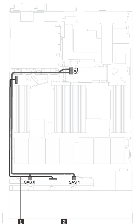
圖例 27. 配備八個 2.5 吋 SAS/SATA 硬碟和一個 8i HBA/RAID 配接卡之伺服器型號的纜線佈線
