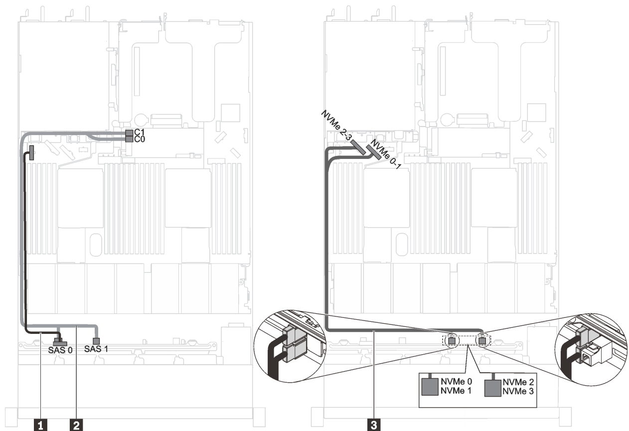
圖例 32. 配備六個 2.5 吋 SAS/SATA 硬碟、四個 2.5 吋 NVMe 硬碟和一個 8i HBA/RAID 配接卡之伺服器型號的纜線佈線
