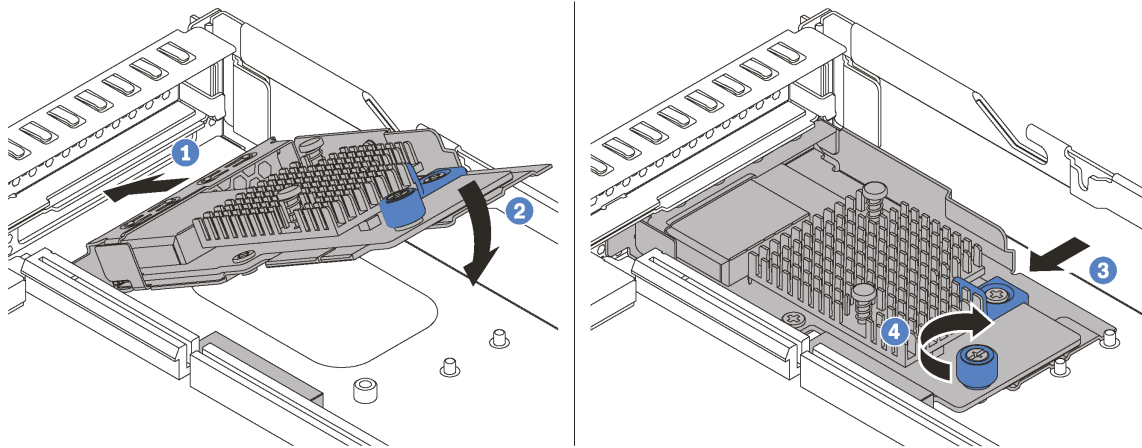
圖例 68. 安裝 LOM 配接卡
