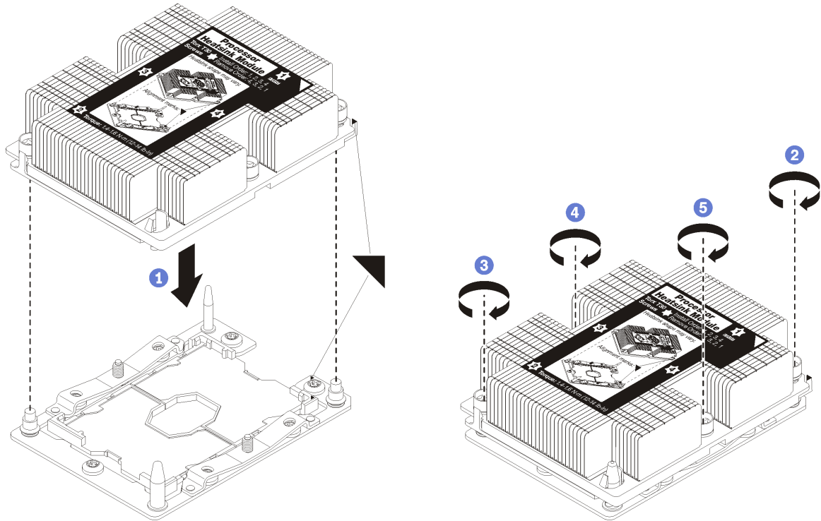
圖例 50. 安裝 PHM
