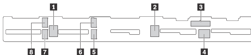
圖例 30. 10 個 2.5 吋 SAS/SATA/NVMe 硬碟背板上的接頭
