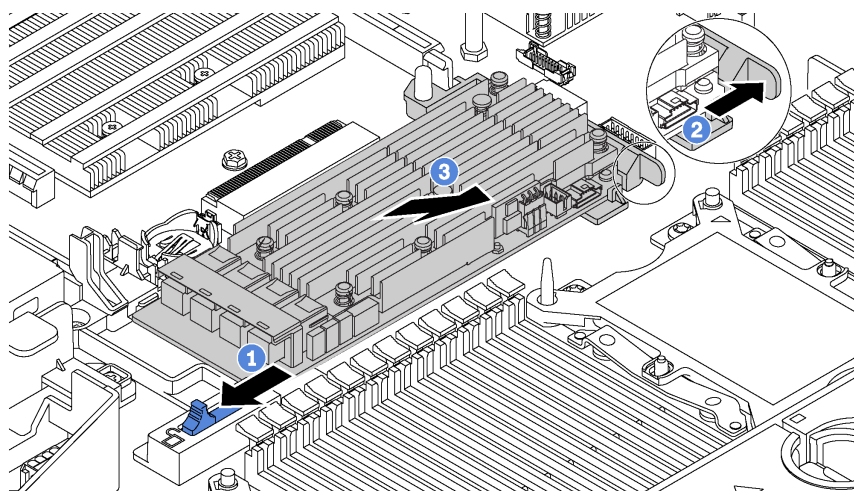
圖例 76. 卸下 RAID 配接卡
