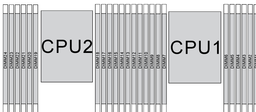
圖例 54. 主機板上的記憶體模組插槽
