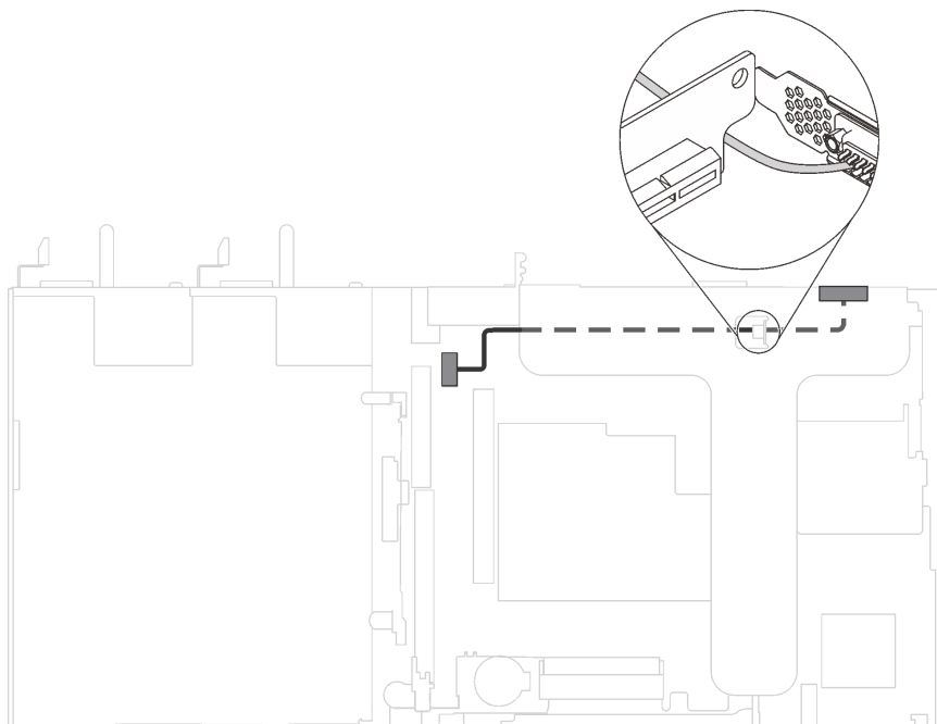
圖例 80. 安裝在 PCIe 插槽 1 中的序列埠模組的纜線佈線
