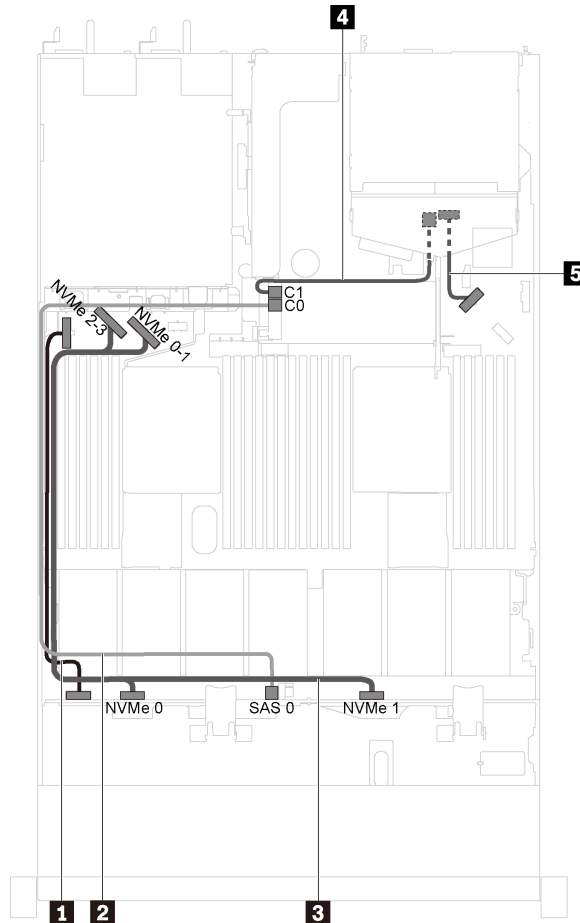
圖例 23. 配備四個 3.5 吋 SAS/SATA/NVMe 硬碟和背面硬碟組件之伺服器型號的纜線佈線
