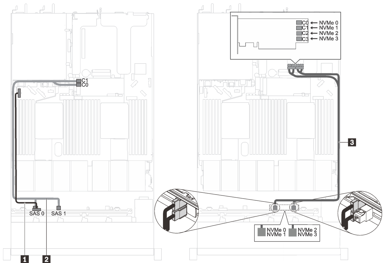
圖例 34. 配備六個 2.5 吋 SAS/SATA 硬碟、四個 2.5 吋 NVMe 硬碟、一個 8i HBA/RAID 配接卡和一個 1610-4P NVMe 交換器配接卡 (在 PCIe 插槽 2 中) 之伺服器型號的纜線佈線
