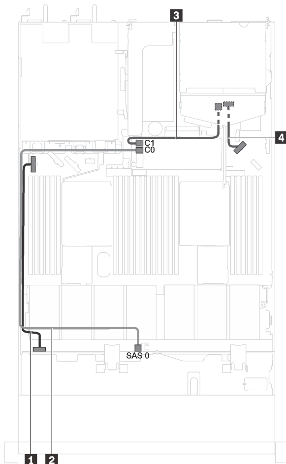
圖例 20. 配備四個 3.5 吋 SAS/SATA 硬碟和背面硬碟組件之伺服器型號的纜線佈線
