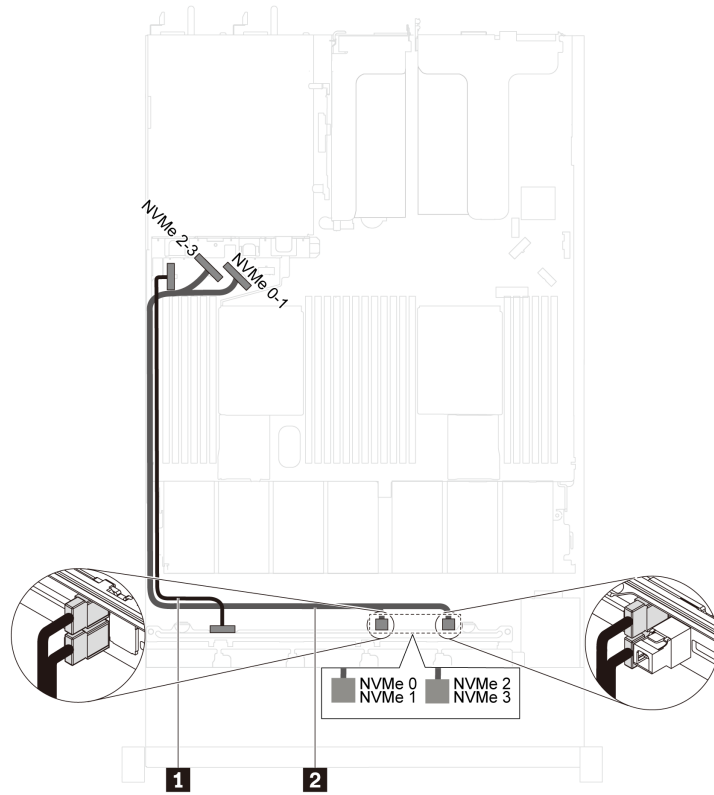
圖例 37. 配備四個 2.5 吋 NVMe 硬碟且無 RAID 配接卡之伺服器型號的纜線佈線
