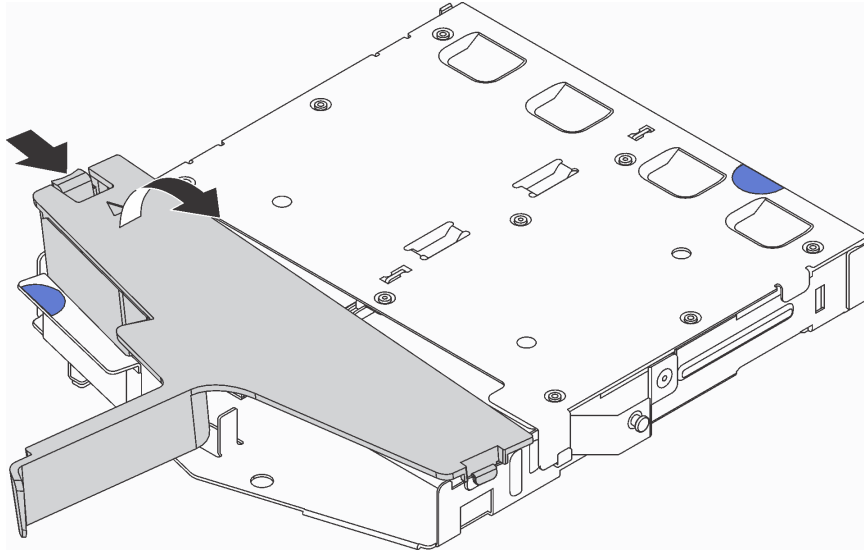
圖例 59. 卸下空氣擋板
