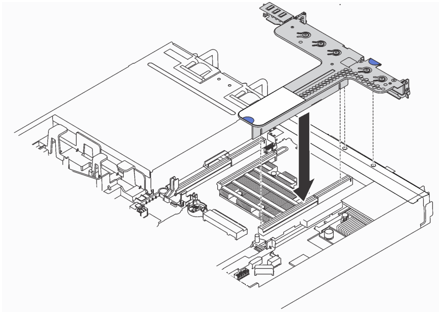
圖例 75. 安裝擴充卡組件
