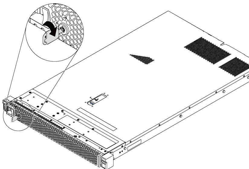
圖例 46. 安全擋板解除鎖定
