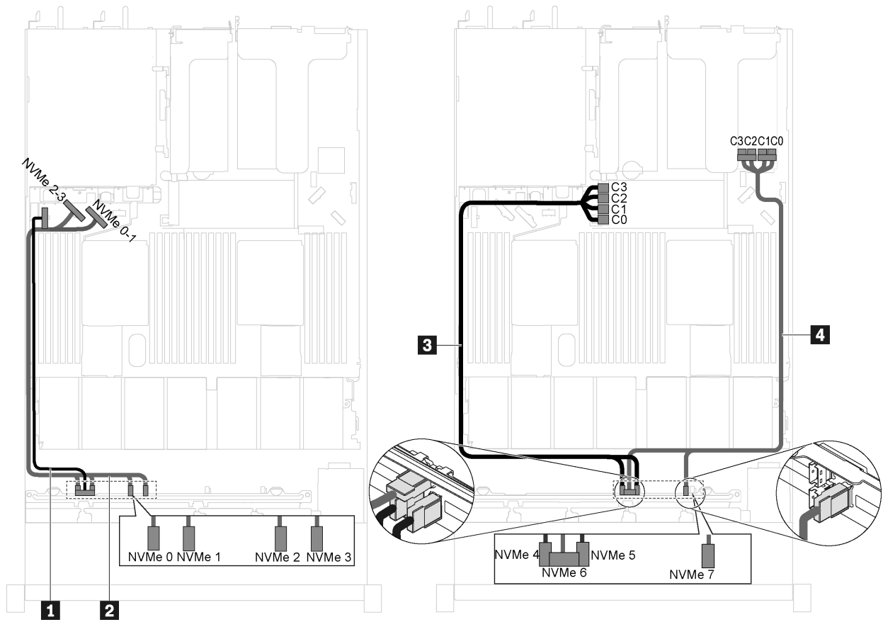
圖例 43. 配備八個 2.5 吋 NVMe 硬碟、一個 810-4P NVMe 交換器配接卡 ( 在 PCIe 插槽 1 中 ) 以及一個 810-4P NVMe 交換器配接卡 ( 在 RAID 配接卡插槽中 ) 之伺服器型號的纜線佈線
