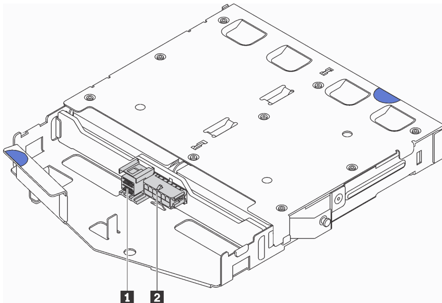
圖例 60. 後方背板接頭
