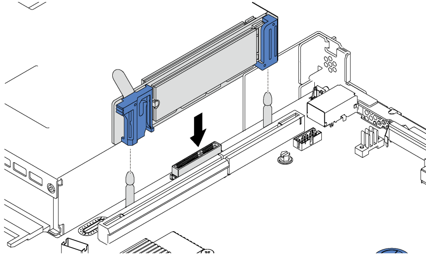
圖例 66. M.2 背板安裝
