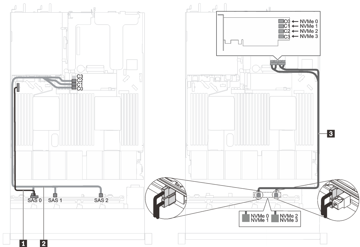
圖例 36. 配備六個 2.5 吋 SAS/SATA 硬碟、四個 2.5 吋 NVMe 硬碟、一個 16i HBA/RAID 配接卡和一個 1610-4P NVMe 交換器配接卡 (在 PCIe 插槽 2 中) 之伺服器型號的纜線佈線
