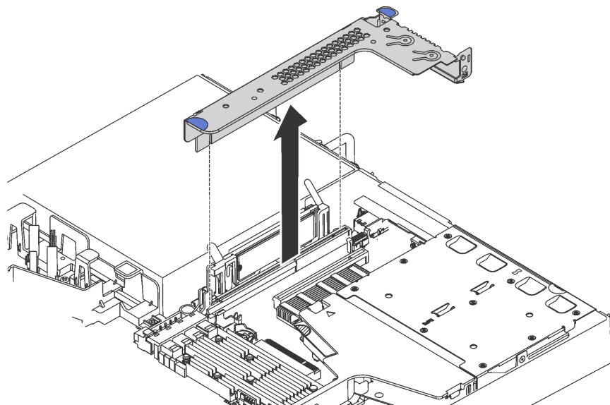
圖例 78. 卸下擴充卡組件
