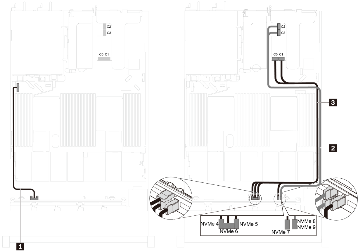
圖例 41. 配備十個 2.5 吋 NVMe 硬碟和一個 NVMe 1611-8P 交換器配接卡 ( 在 PCIe 插槽 2 中 ) 之伺服器型號的纜線佈線
