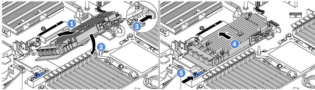
圖例 58. 安裝 RAID 配接卡
