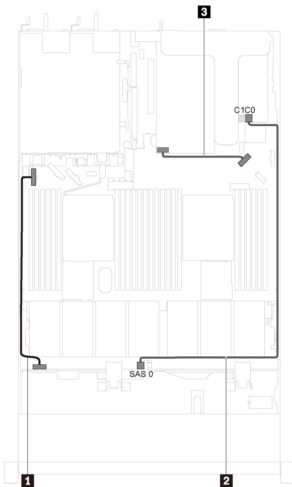
圖例 21. 配備四個 3.5 吋 SAS/SATA 硬碟和全高半長 GPU 之伺服器型號的纜線佈線
