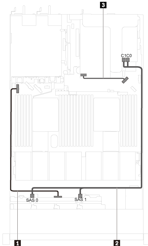
圖例 29. 配備八個 2.5 吋 SAS/SATA 硬碟和全高半長 GPU 之伺服器型號的纜線佈線
