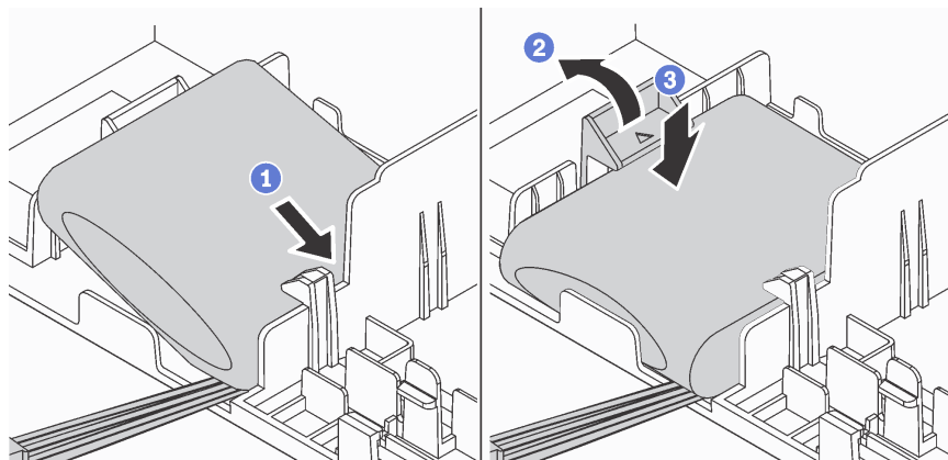
圖例 82. 將 RAID 超級電容器模組安裝在空氣擋板的底端
