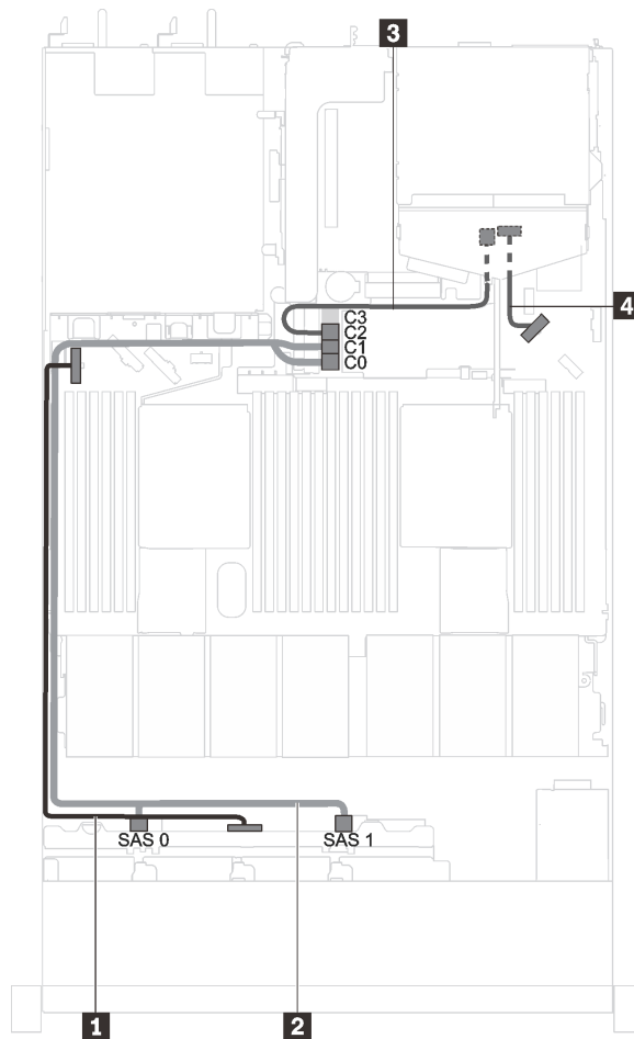
圖例 28. 配備八個 2.5 吋 SAS/SATA 硬碟、一個 16i HBA/RAID 配接卡和背面硬碟組件之伺服器型號的纜線佈線
