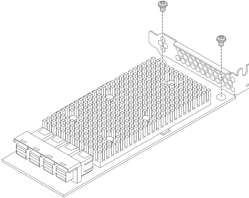
圖例 77. 將半高托架安裝到 RAID 配接卡
