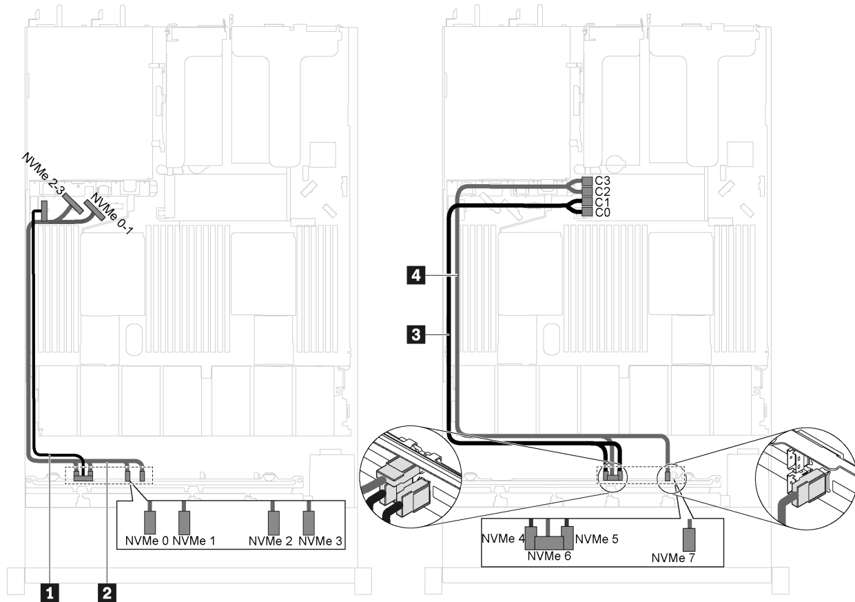
圖例 42. 配備八個 2.5 吋 NVMe 硬碟和一個 810-4P NVMe 交換器配接卡 ( 在 RAID 配接卡插槽中 ) 之伺服器型號的纜線佈線
