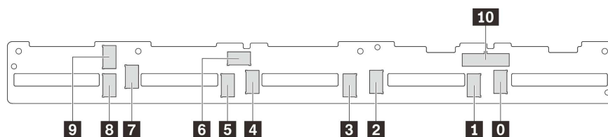
圖例 38. 10 個 2.5 吋 NVMe 硬碟背板上的接頭
