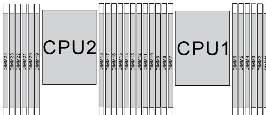
圖例 53. 主機板上的記憶體模組插槽
