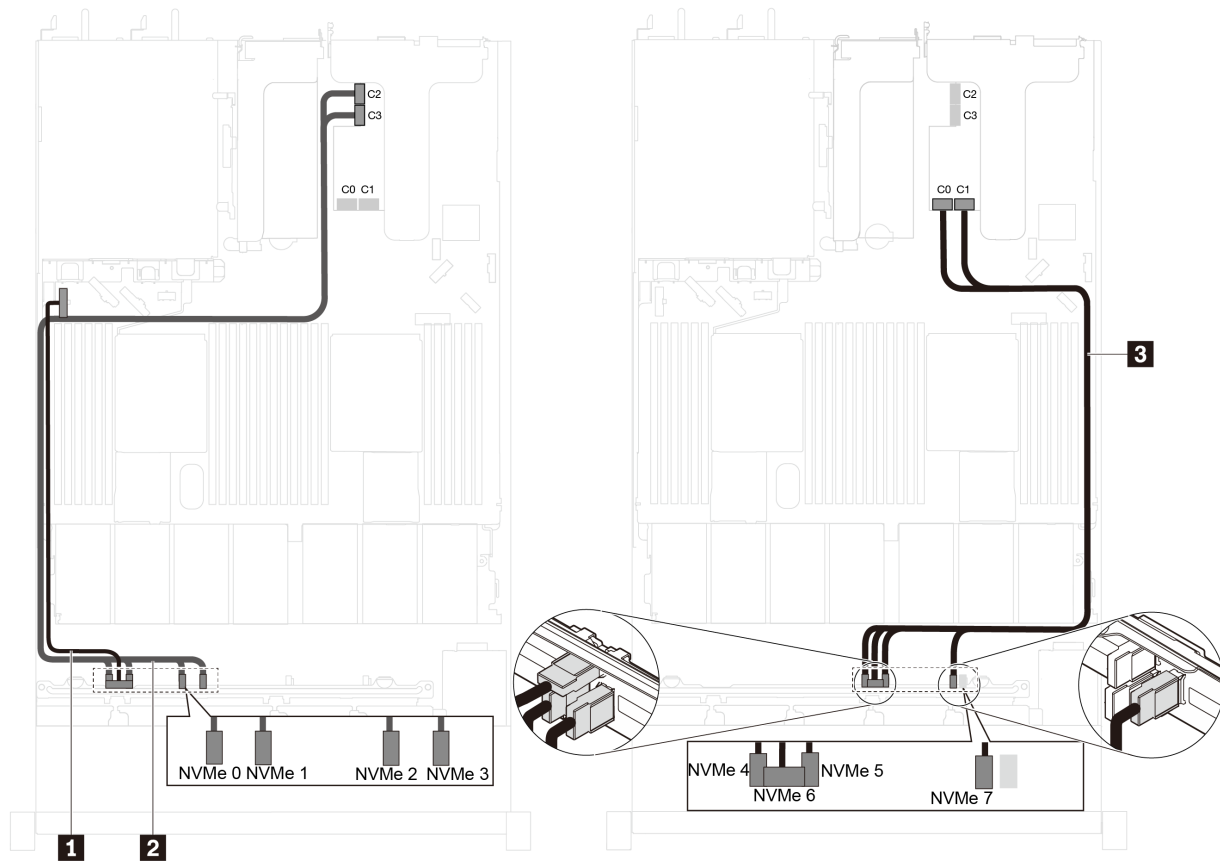
圖例 44. 配備八個 2.5 吋 NVMe 硬碟和一個 NVMe 1611-8P 交換器配接卡 ( 在 PCIe 插槽 2 中 ) 之伺服器型號的纜線佈線
