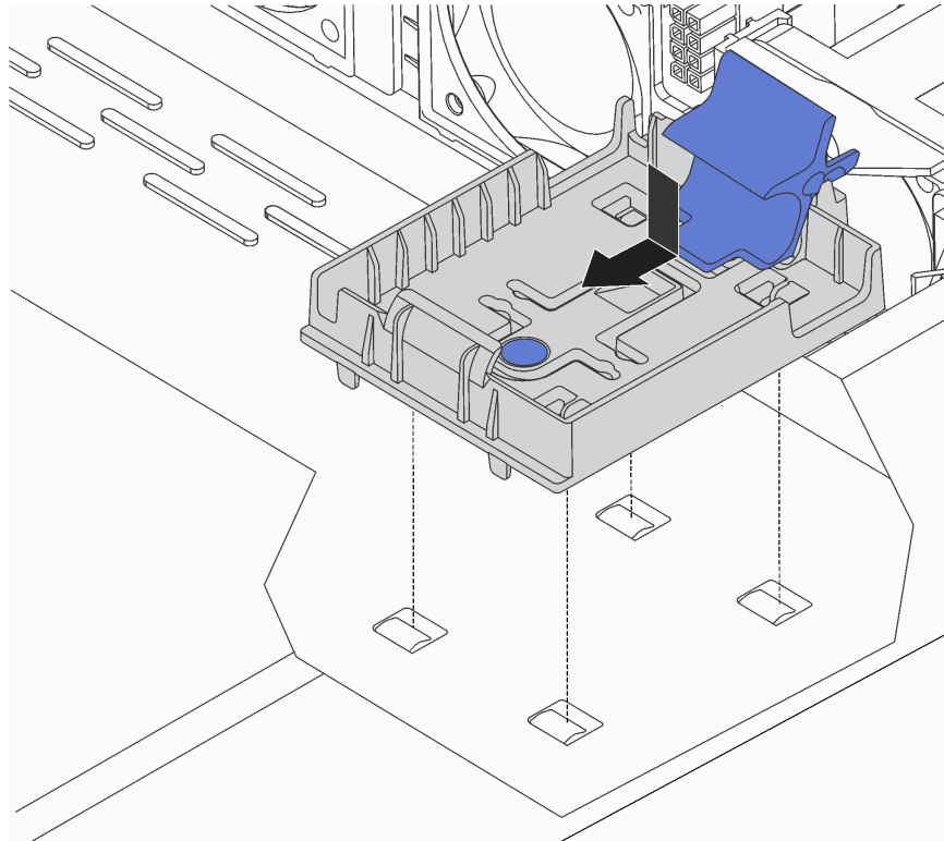
圖例 85. 安裝 RAID 超級電容器模組匣
