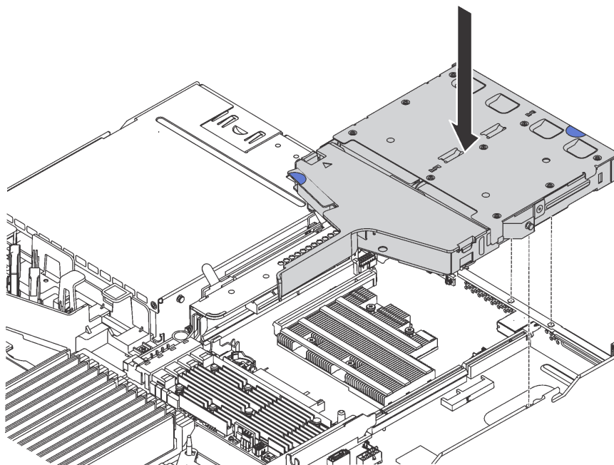
圖例 62. 安裝背面熱抽換硬碟組件
