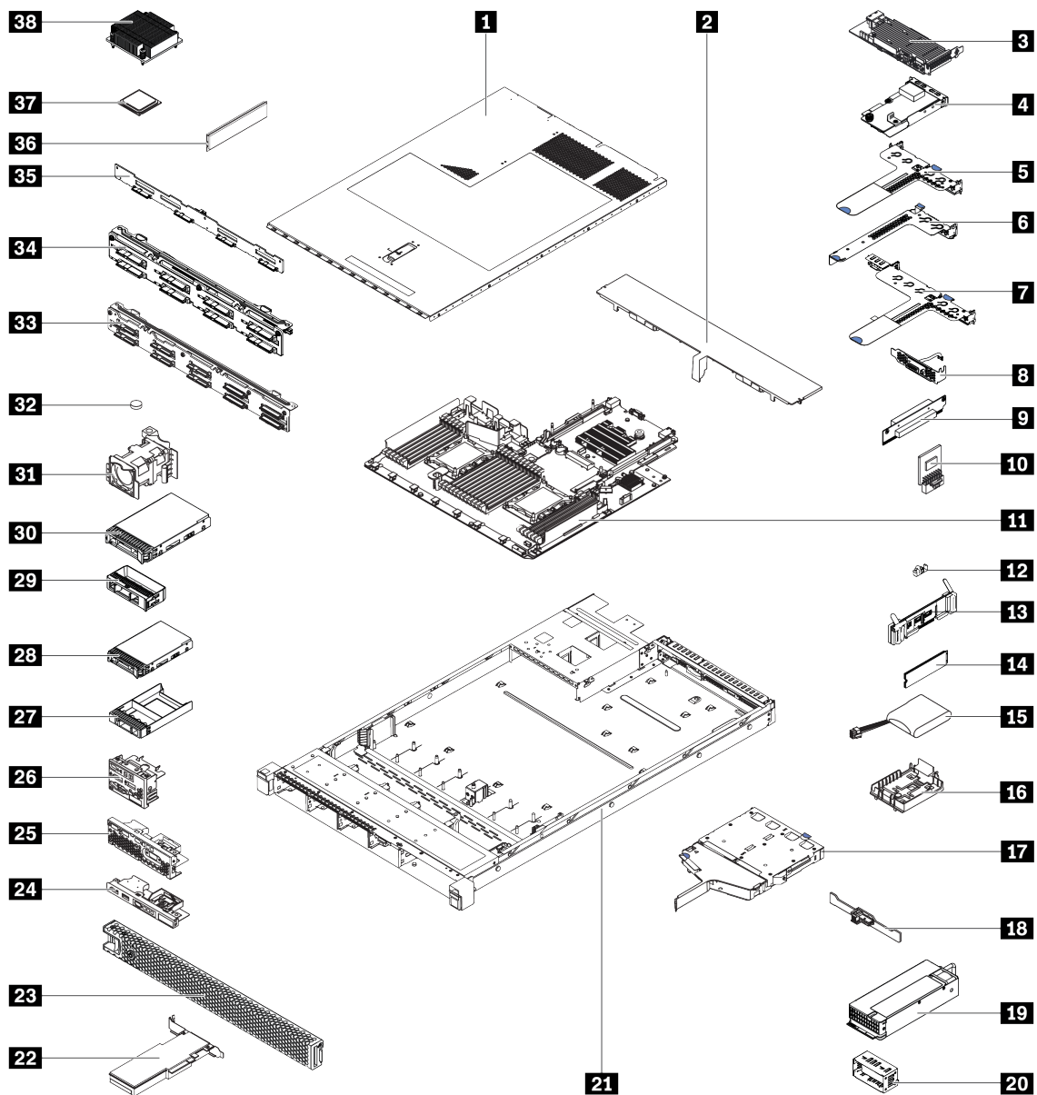
圖例 45. 伺服器元件
