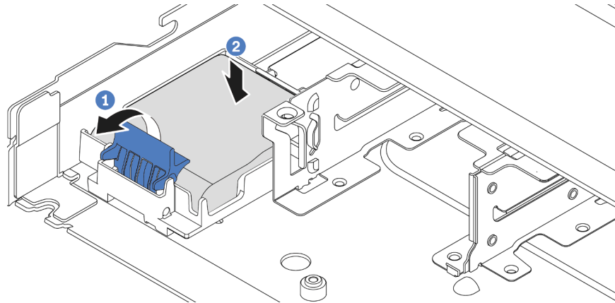
Figura 113. Instalación del módulo de alimentación flash RAID en la bandeja de la placa del sistema
