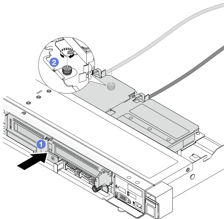
Figura 24. Instalación del compartimiento de expansión frontal
