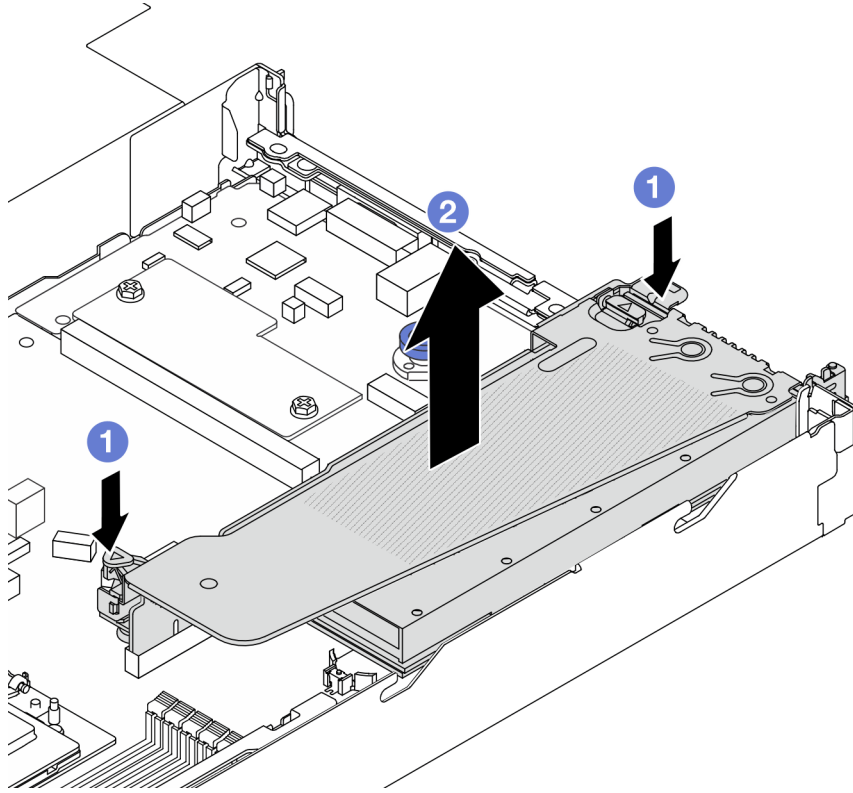
Figura 47. Extracción del conjunto de expansión
