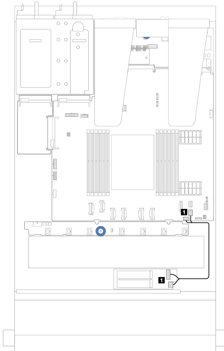
Figura 220. Disposición de los cables de SATA
