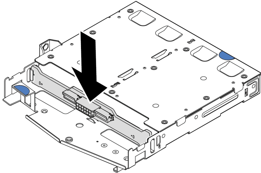
Figura 7. Instalación de la placa posterior
