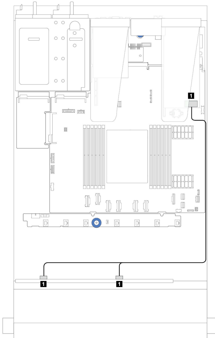
Figura 236. Disposición de los cables para 8 bahías de unidades SAS/SATA frontales de 2,5" con un adaptador RAID SFF 8i o 16i (Gen 4)
