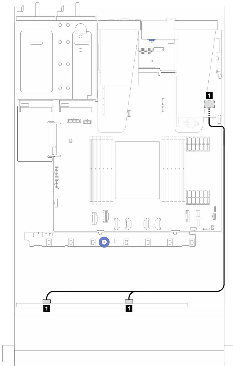
Figura 240. Disposición de los cables para 8 unidades U.3 frontales de 2,5" con un adaptador RAID SFF 8i (Gen 4)
