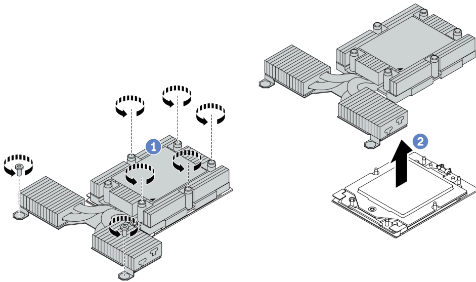
Figura 92. Extracción de un disipador de calor de refrigeración de aire
