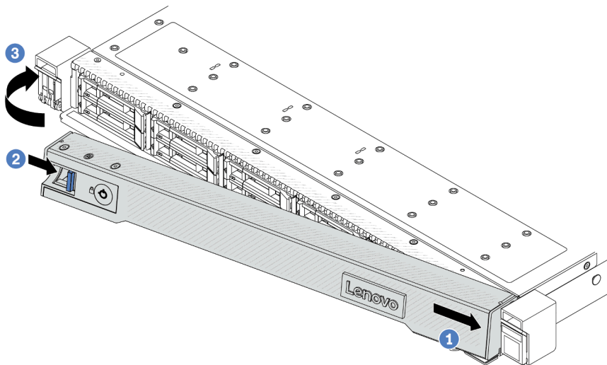
Figura 169. Instalación del marco biselado de seguridad
