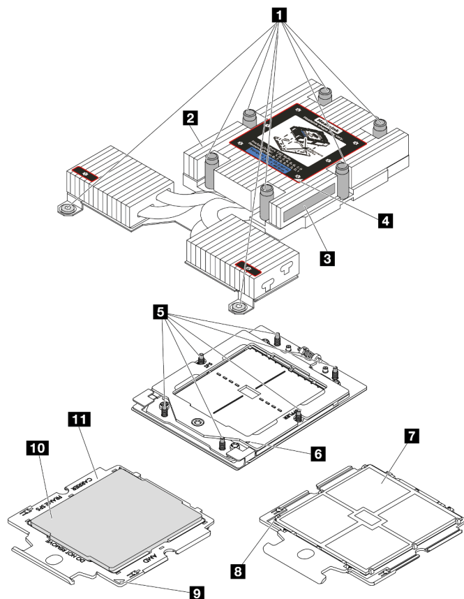
Figura 91. Componentes del procesador y el disipador de calor
