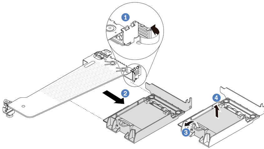
Figura 114. Extracción del módulo de alimentación flash RAID del conjunto de expansión
