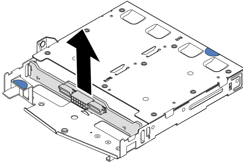
Figura 6. Extracción de la placa posterior de la unidad posterior de 2,5 pulgadas
