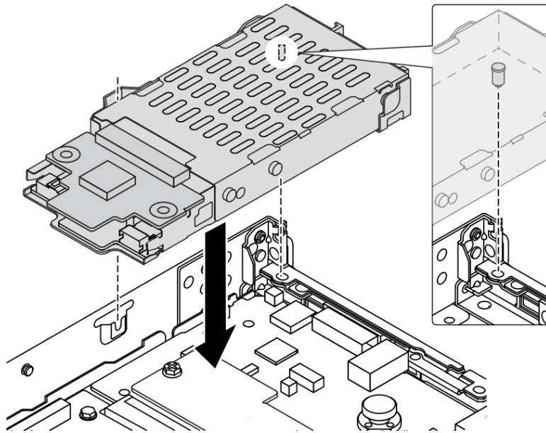
Figura 165. Instalación del compartimiento de unidad de intercambio en caliente posterior
