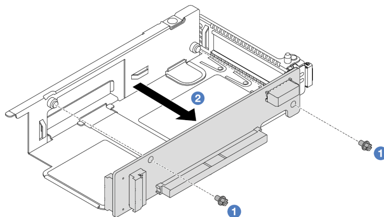
Figura 27. Extracción de la tarjeta de expansión del compartimiento de bajo perfil
