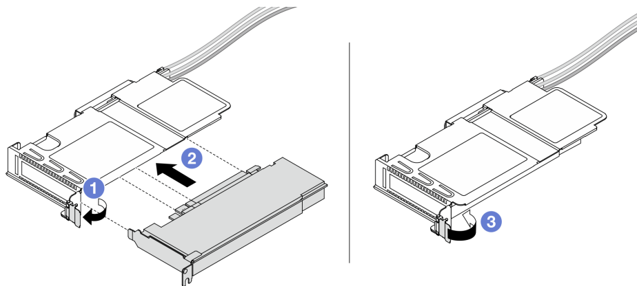
Figura 31. Instalación del adaptador PCIe
