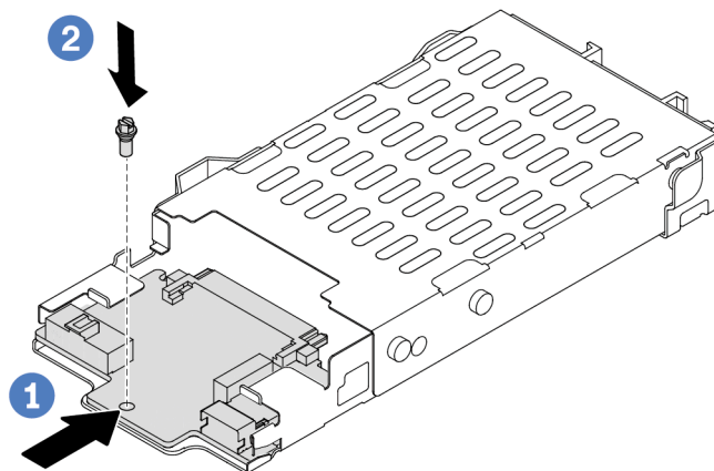
Figura 11. Instalación de la placa posterior de la unidad de 7 mm (inferior)
