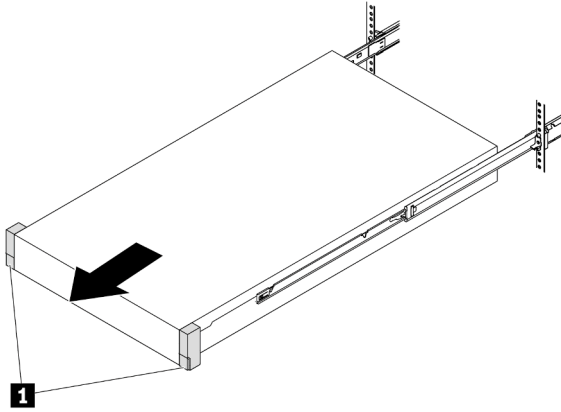
Figura 52. Extracción del servidor
