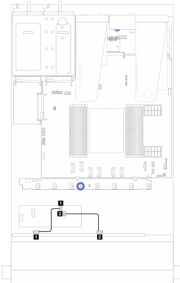
Figura 239. Disposición de los cables para 8 bahías de unidades SAS/SATA frontales de 2,5" con un adaptador RAID/HBA CFF 8i (Gen 3)
