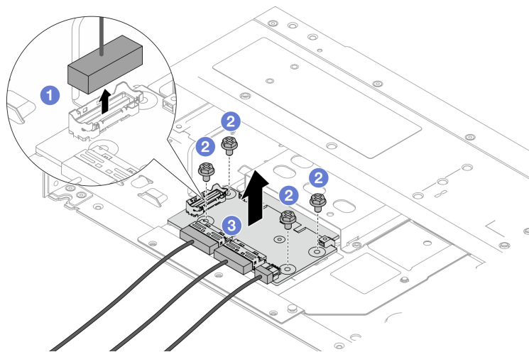
Figura 35. Extracción de la tarjeta de interposición de OCP frontal
