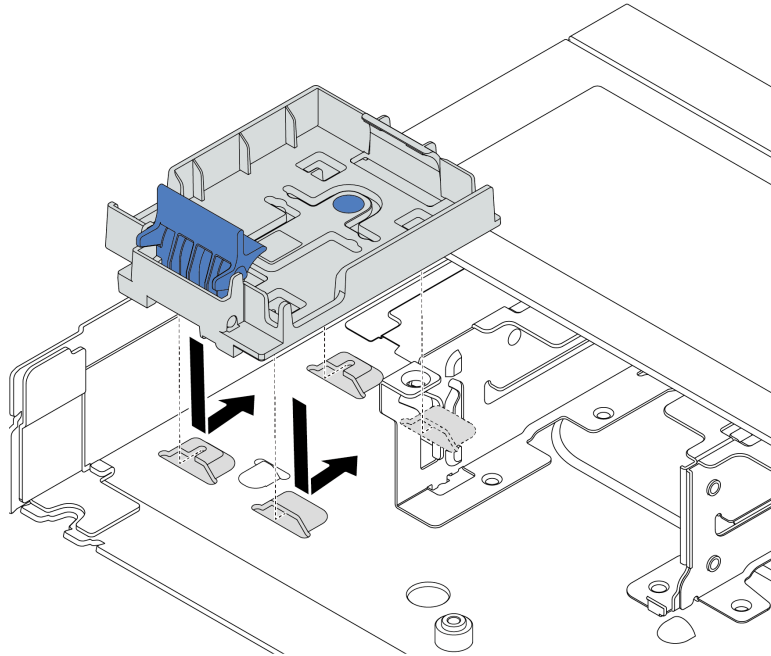
Figura 107. Instalación del compartimento del módulo de alimentación flash RAID
