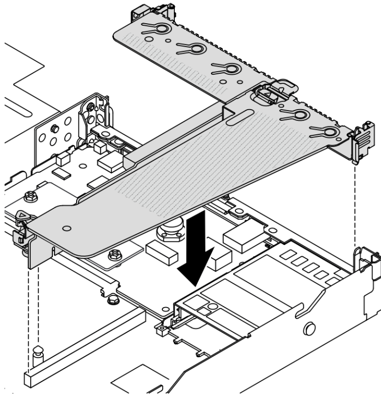
Figura 152. Instalación del conjunto de expansión
