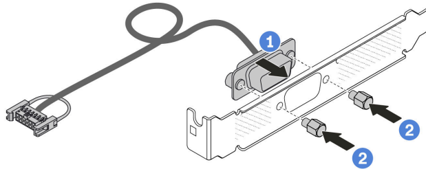
Figura 174. Ensamblaje del módulo de puerto serie
