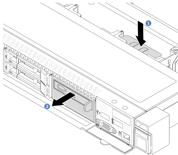
Figura 40. Extracción del conjunto del panel de diagnóstico integrado
