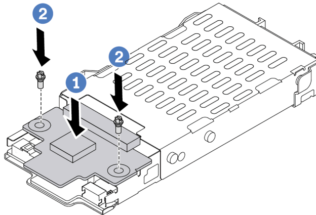
Figura 12. Instalación de la placa posterior de 7 mm (superior)
