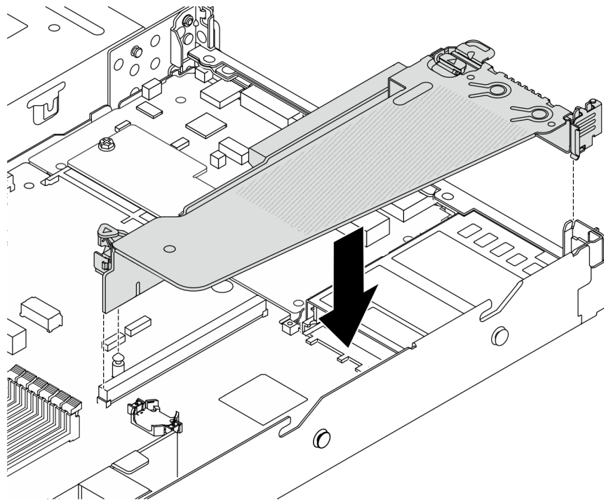
Figura 176. Instalación del conjunto de expansión
