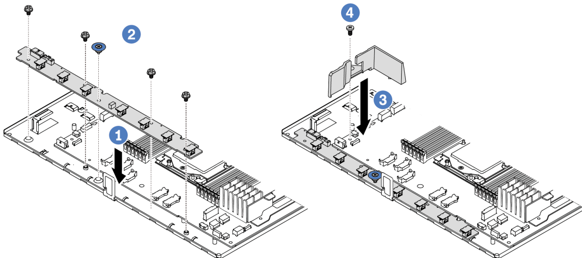
Figura 46. Instalación de la placa del ventilador
