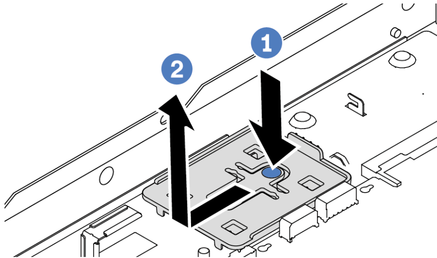
Figura 111. Extracción de la bandeja
