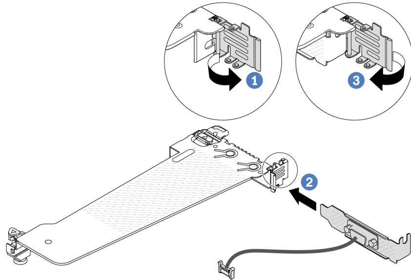
Figura 175. Instalación del módulo de puerto serie
