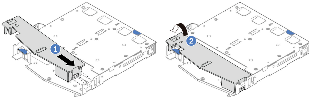
Figura 8. Instalación del deflector de aire
