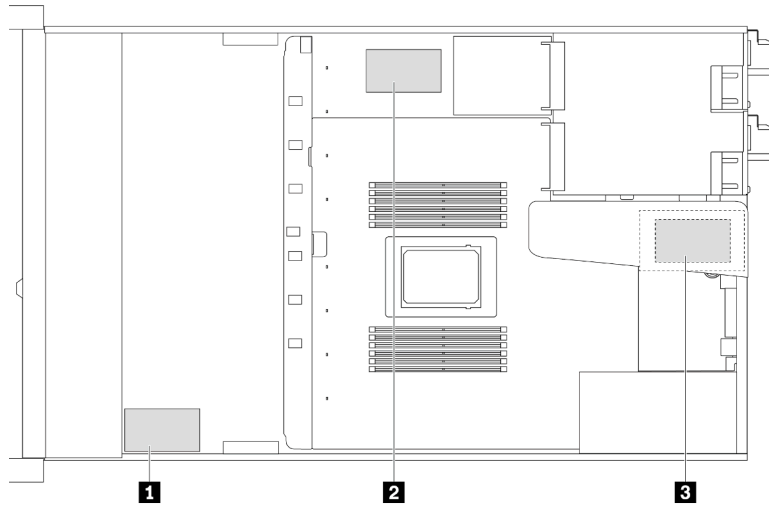
Figura 206. Módulos de alimentación flash RAID en el chasis
