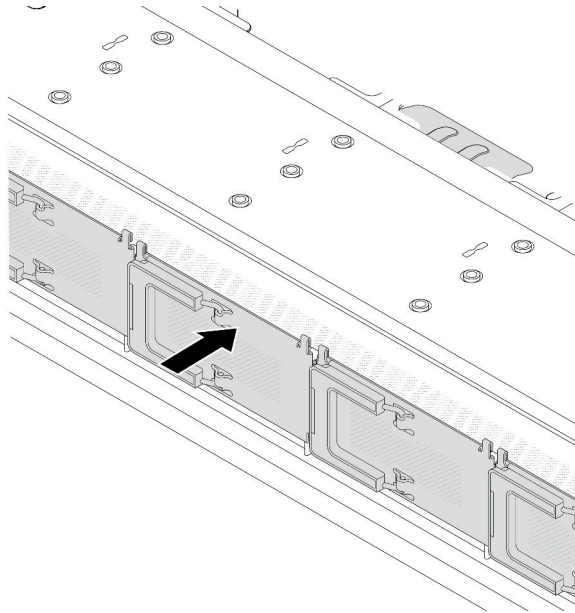
Figura 66. Instalación de la cubierta del compartimiento de la unidad EDSFF
