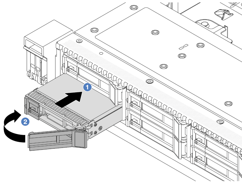
Figura 61. Instalación de unidad de intercambio en caliente
