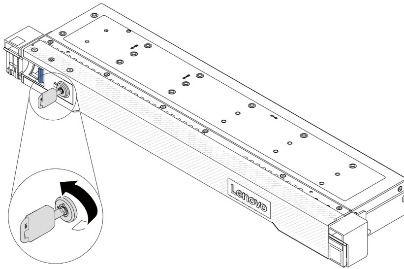
Figura 170. Bloqueo del marco biselado de seguridad
