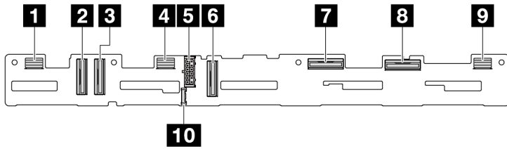
Figura 192. Placa posterior de 10 unidades AnyBay de 2,5" (Gen 5)
