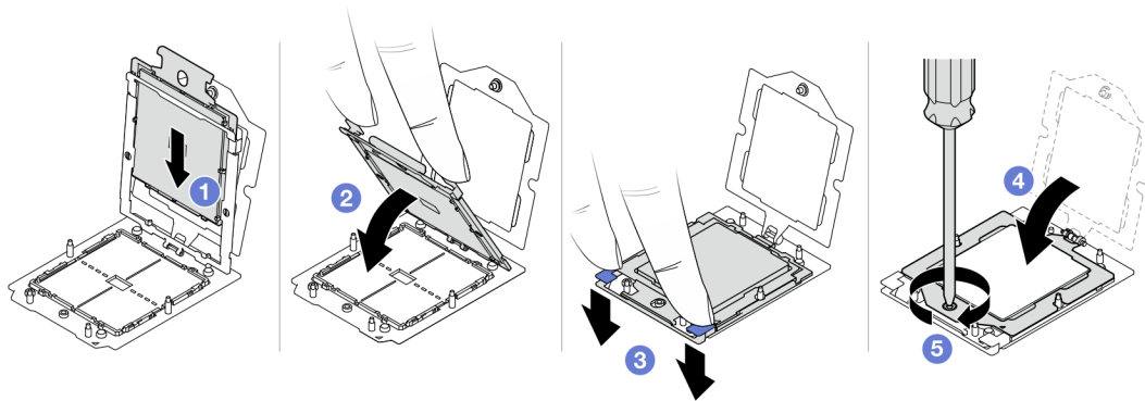
Figura 96. Instalación de un procesador
