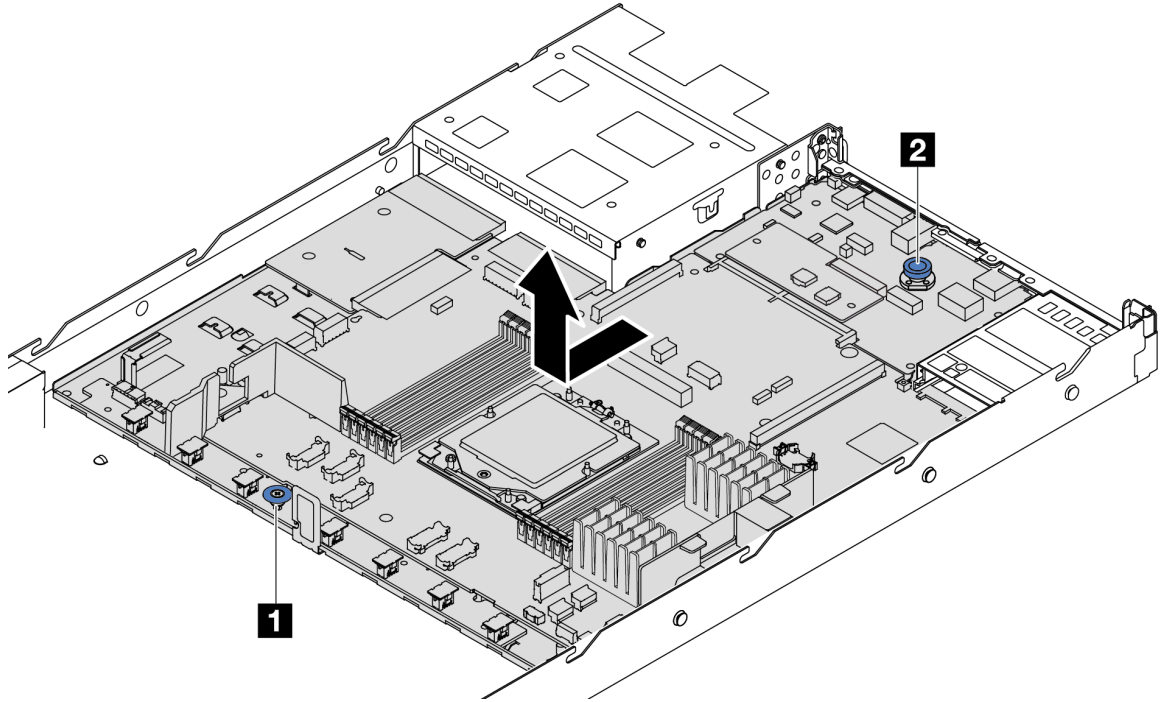
Figura 181. Extracción del conjunto de la placa del sistema
