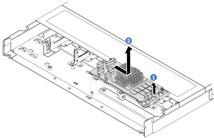
Figura 72. Extracción del adaptador HBA/RAID CFF interno
