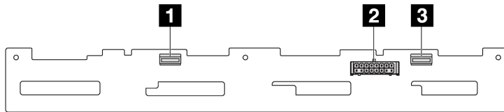
Figura 193. 8 placas posteriores SAS/SATA de 2,5"
