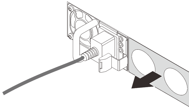
Figura 70. Extracción de relleno de fuente de alimentación de intercambio en caliente
