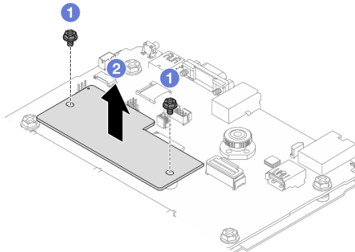
Figura 178. Extracción del Firmware y módulo de seguridad de RoT
