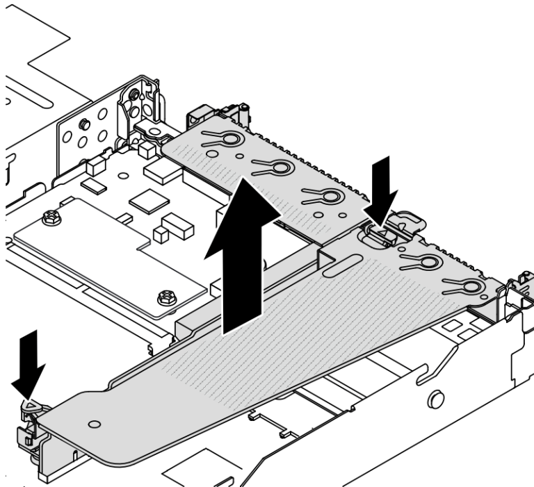
Figura 148. Extracción del conjunto de expansión
