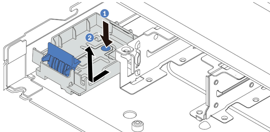
Figura 105. Extracción del compartimento del módulo de alimentación flash RAID
