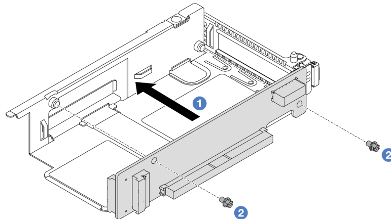
Figura 29. Instalación de la tarjeta de expansión en un compartimiento de bajo perfil
