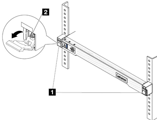
Figura 59. Fijación del servidor en la parte frontal del bastidor
