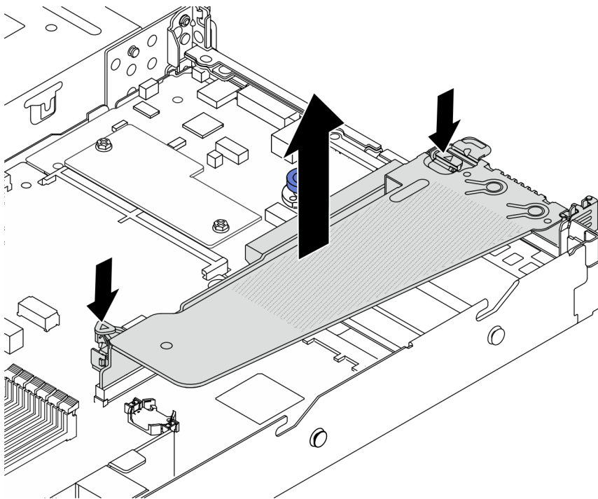
Figura 171. Extracción de la abrazadera de expansión
