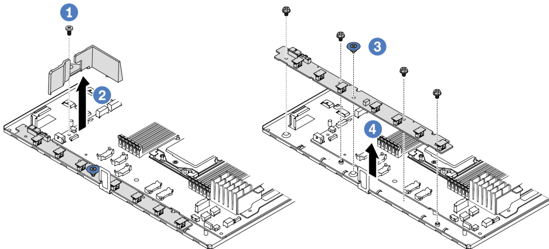
Figura 45. Extracción de la placa de ventilador
