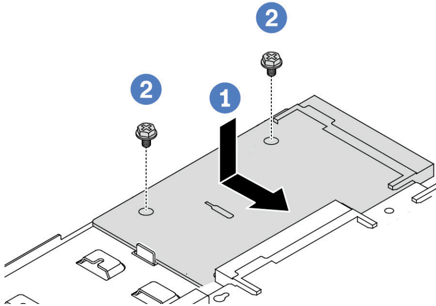
Figura 98. Instalación de la placa PIB
