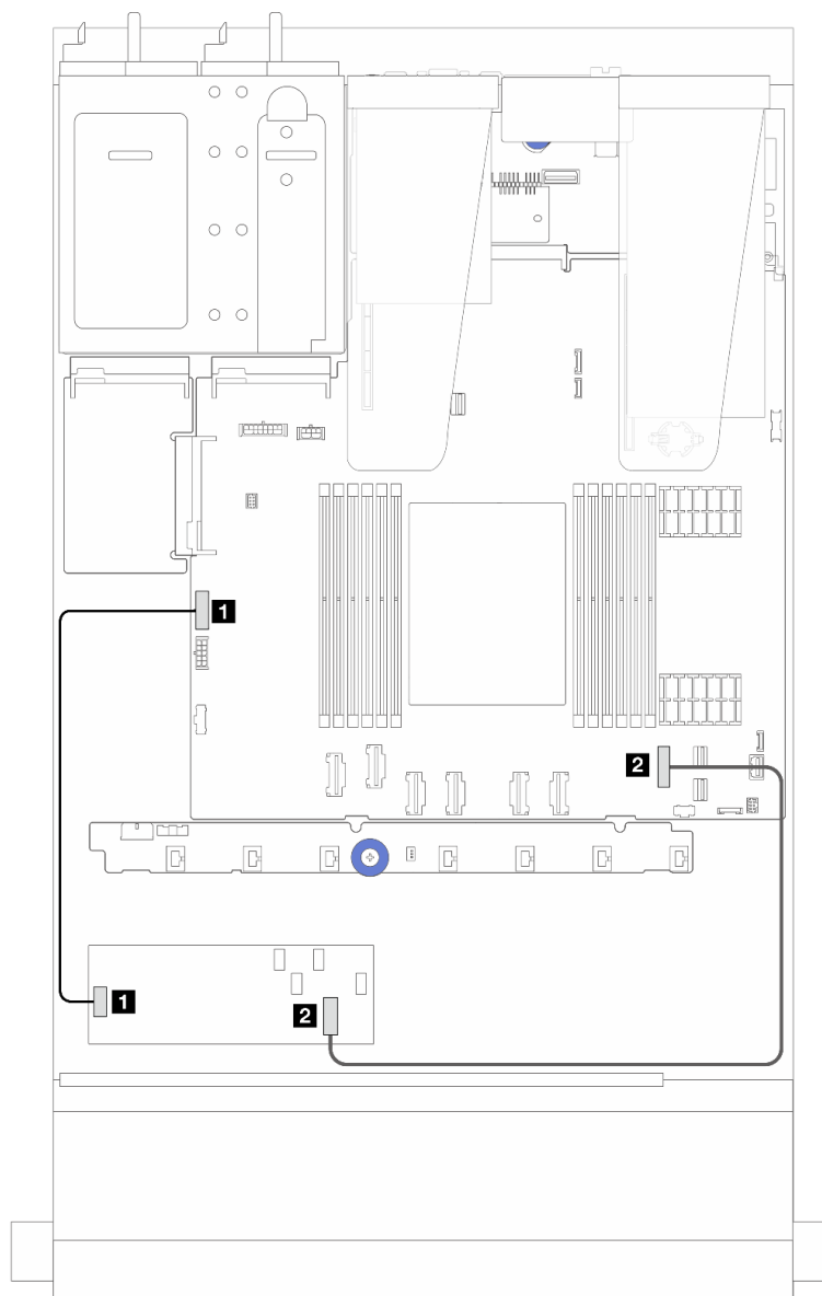
Figura 201. Cableado de alimentación y de entrada del adaptador Gen 4 CFF RAID
