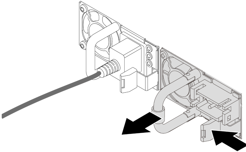
Figura 68. Extracción de la unidad de fuente de alimentación
