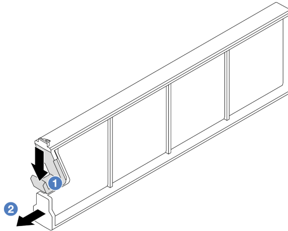
Figura 64. Extracción de un relleno de unidad EDSFF
