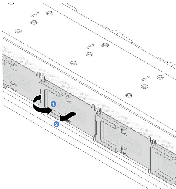
Figura 62. Extracción de la cubierta del compartimiento de la unidad EDSFF
