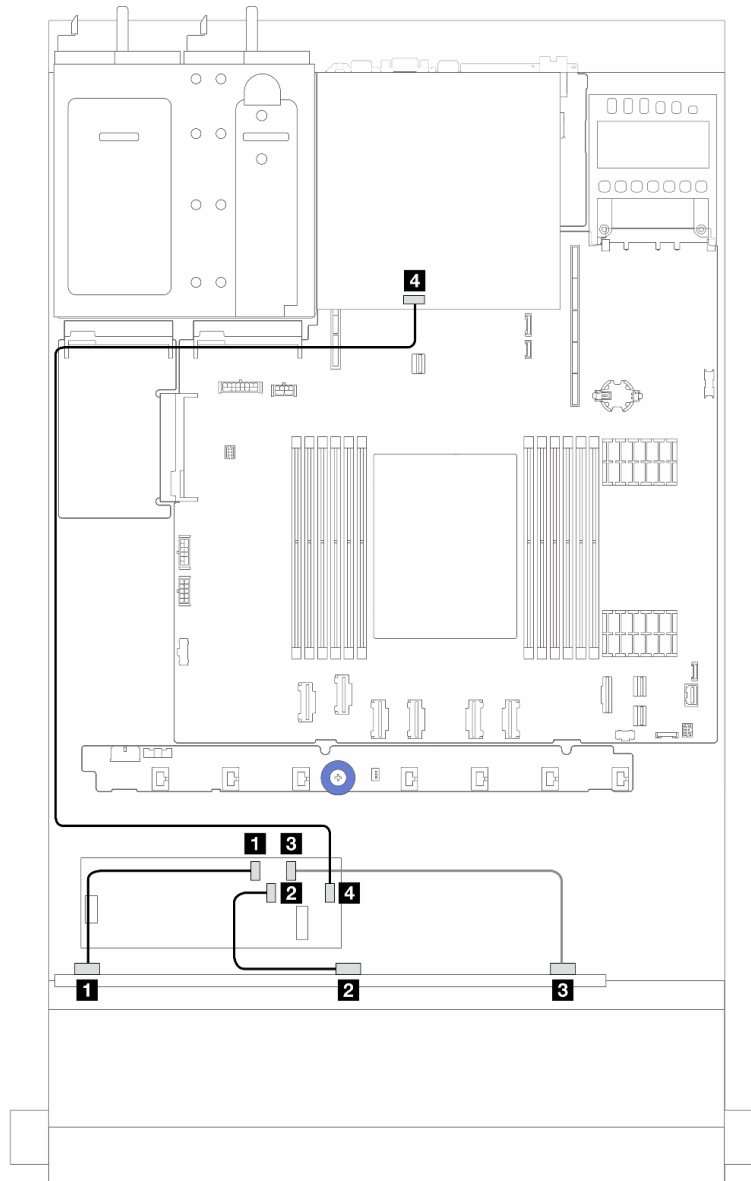
Figura 248. Disposición de los cables para 6 unidades SAS/SATA frontales y 4 bahías de unidades AnyBay frontales y un adaptador RAID CFF 16i (Gen 3 o Gen 4) con 2 unidades SAS/SATA traseras de 2,5" instaladas
