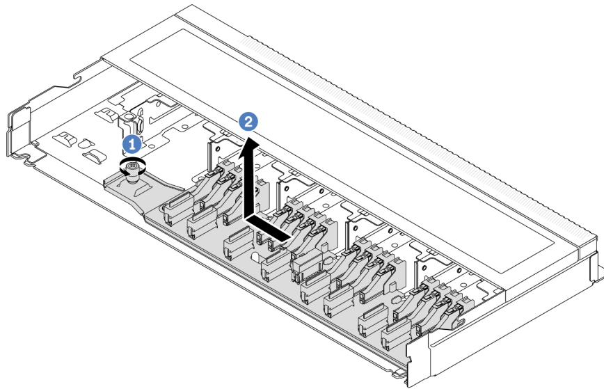
Figura 4. Instalación de la placa posterior para unidades 16 EDSFF
