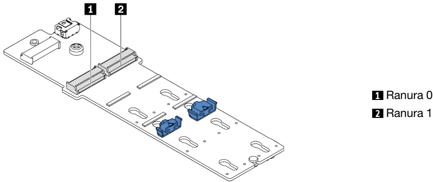
Figura 82. Ranura de unidad M.2
