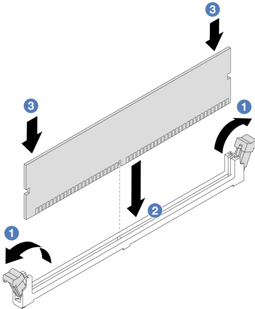
Figura 78. Instalación de un módulo de memoria
