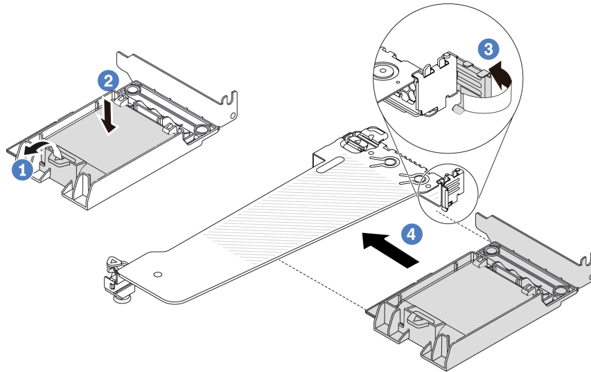
Figura 115. Instalación del módulo de alimentación flash RAID en el conjunto de expansión
