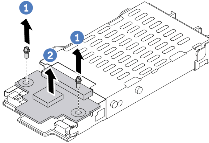
Figura 9. Extracción de la placa posterior de la unidad de 7 mm (superior)
