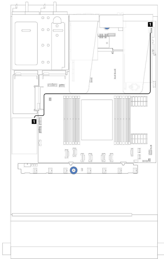
Figura 210. Disposición de los cables de los módulos de alimentación flash RAID en la bandeja de la placa del sistema
