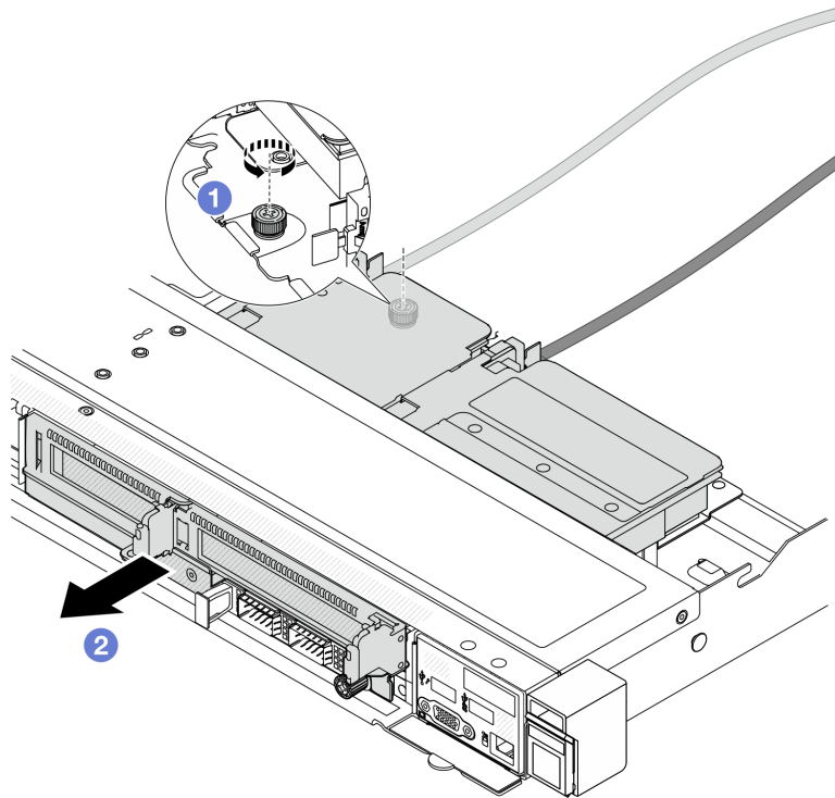
Figura 23. Extracción del compartimiento de expansión frontal
