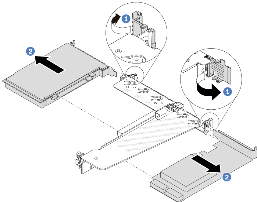
Figura 87. Extracción de un adaptador PCIe del conjunto de expansión LP-FH
