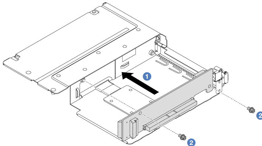
Figura 30. Instalación de la tarjeta de expansión en un compartimiento de altura completa
