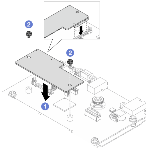
Figura 179. Instalación del Firmware y módulo de seguridad de RoT
