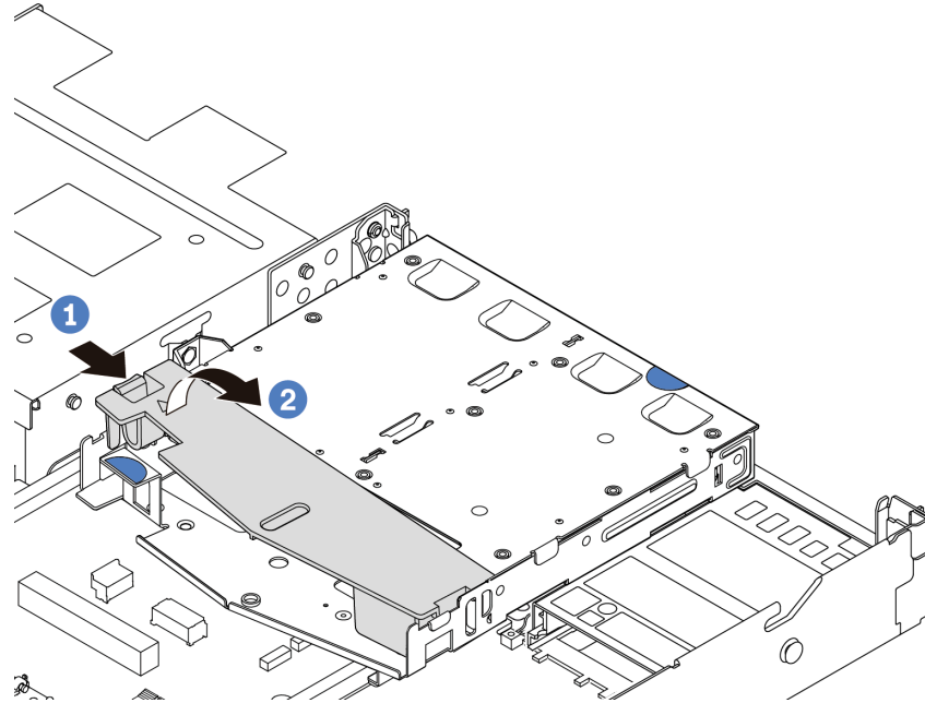
Figura 5. Extracción del deflector de aire
