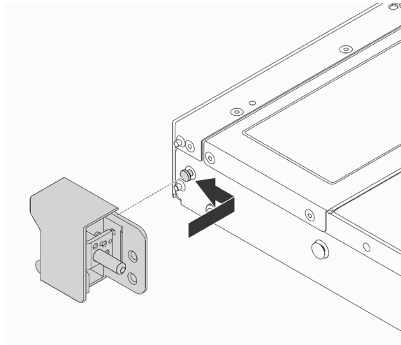
Figura 101. Instalación del pestillo del bastidor
