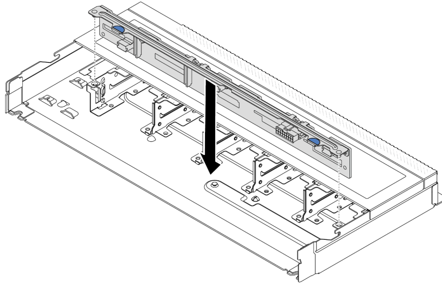
Figura 2. Instalación de la placa posterior de diez unidades de intercambio en caliente de 2,5"
