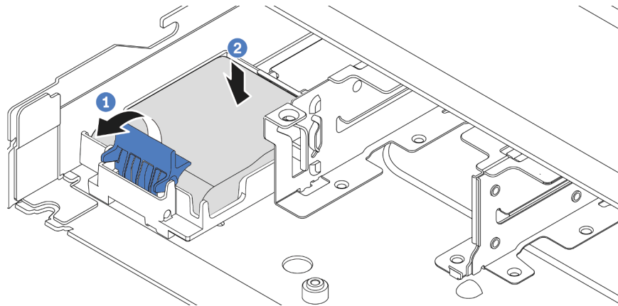
Figura 108. Instalación del módulo de alimentación flash RAID en el chasis
