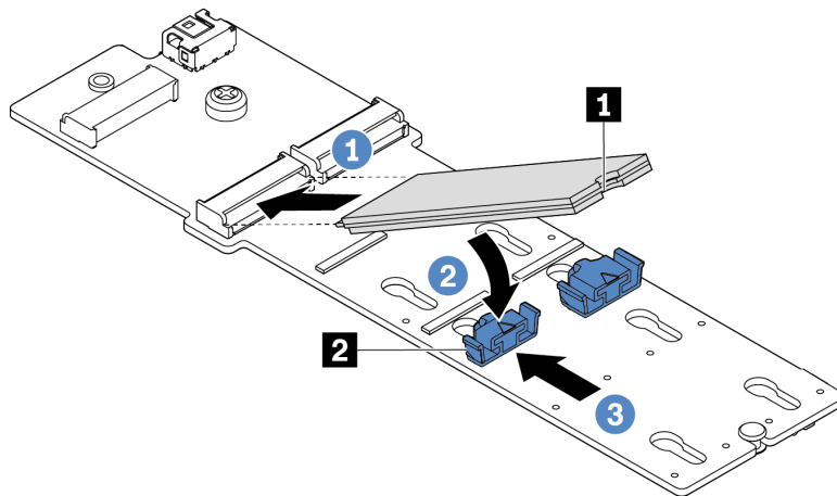
Figura 84. Instalación de la unidad M.2
