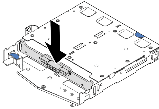
Figura 160. Instalación de la placa posterior
