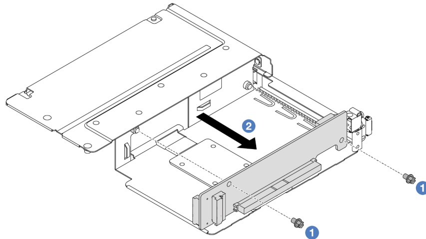
Figura 28. Extracción de la tarjeta de expansión del compartimiento de altura completa
