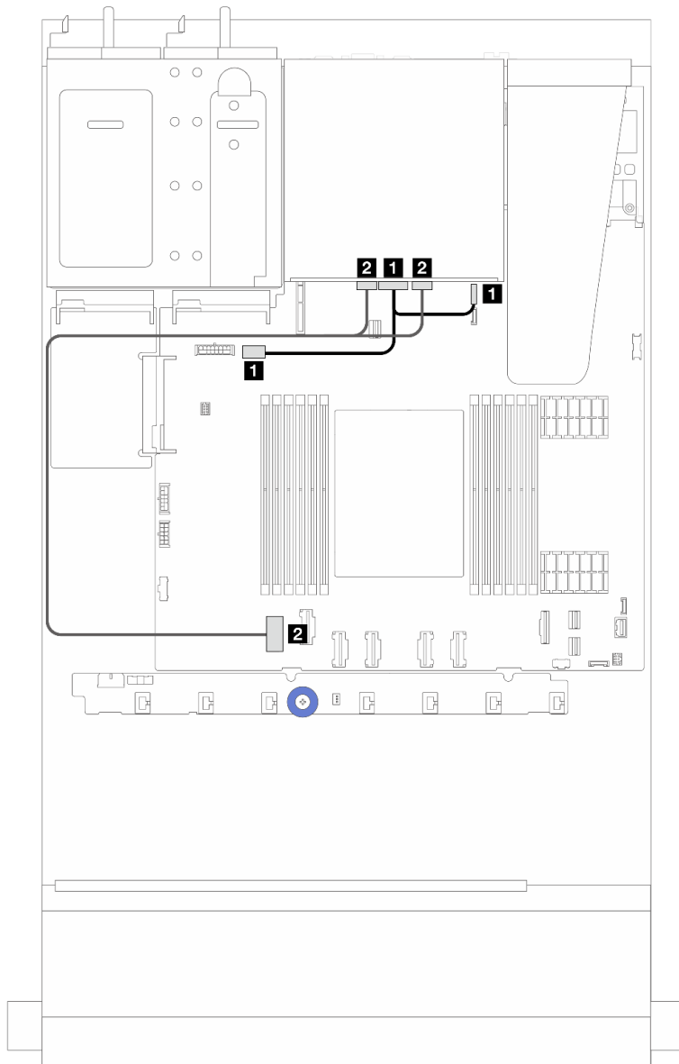
Figura 212. Disposición de los cables de la placa posterior de la unidad NVMe de 2 unidades de 2,5" trasera
