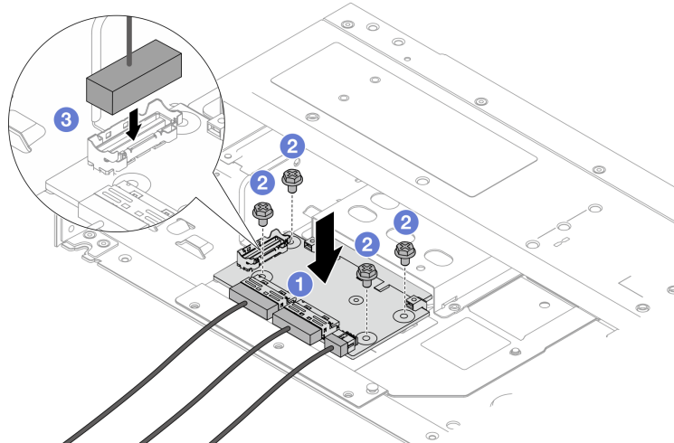
Figura 36. Instalación de la tarjeta de interposición de OCP frontal
