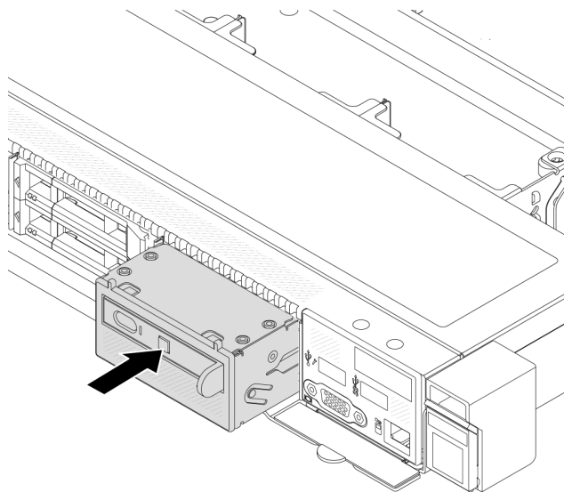
Figura 44. Instalación del conjunto de panel de diagnósticos
