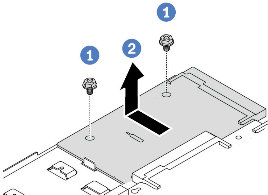
Figura 97. Extracción de la placa PIB
