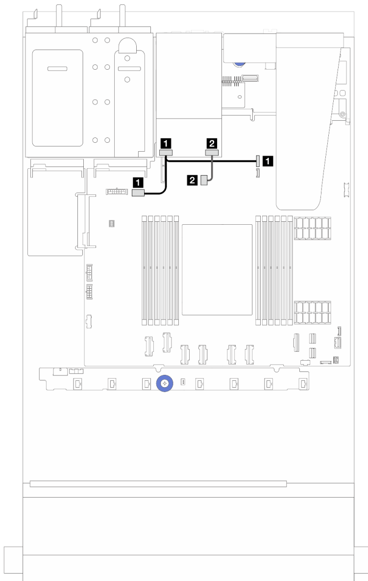
Figura 215. Disposición de los cables NVMe
