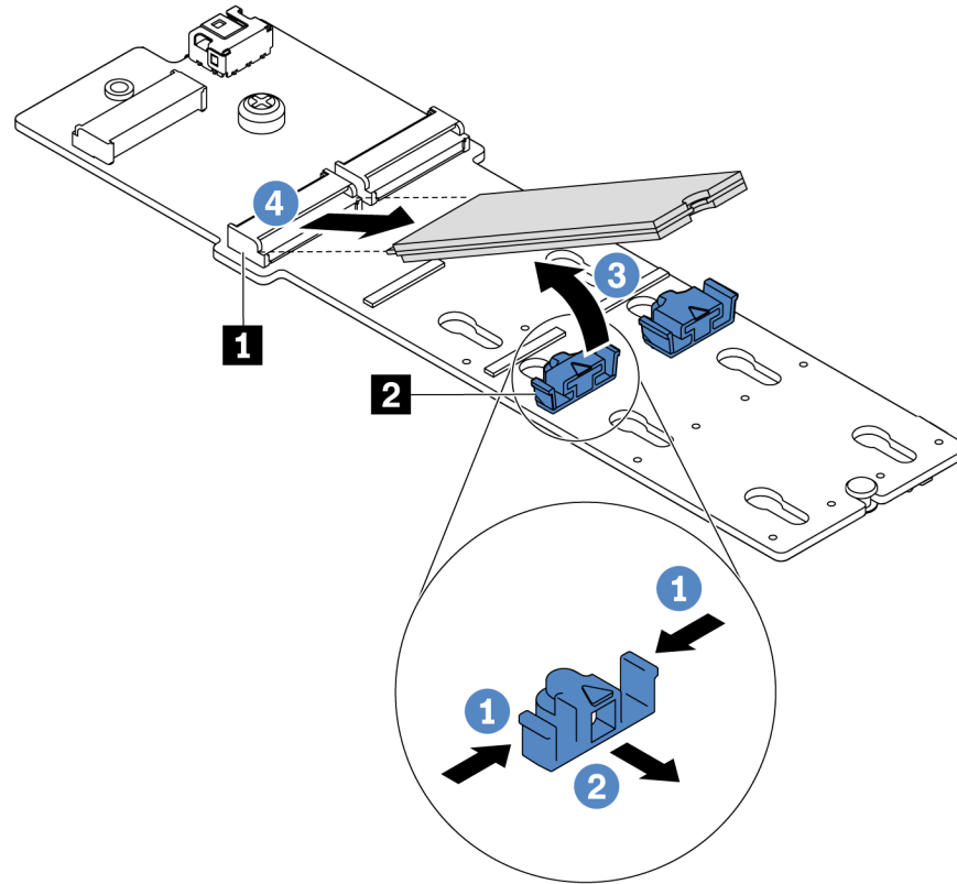
Figura 79. Quitar la unidad M.2
