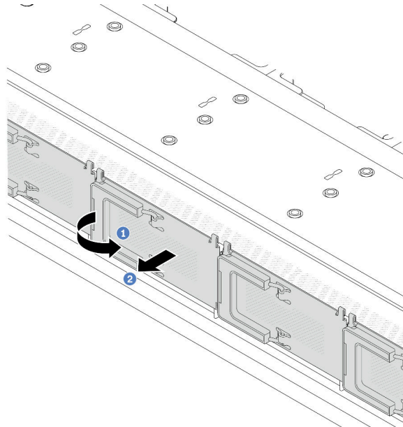
Figura 17. Extracción de la cubierta del compartimiento de la unidad EDSFF
