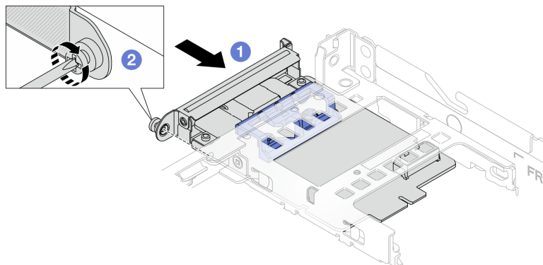
Figura 76. Instalación del adaptador NIC de gestión
