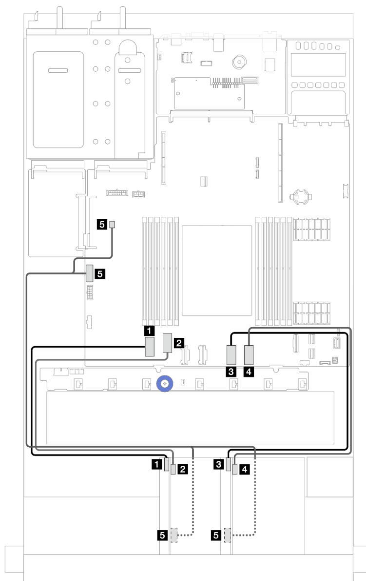
Figura 203. Disposición de los cables para el conjunto de expansión frontal
