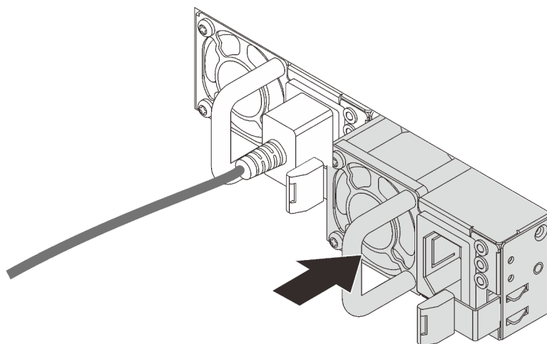
Figura 71. Instalación de una fuente de alimentación de intercambio en caliente
