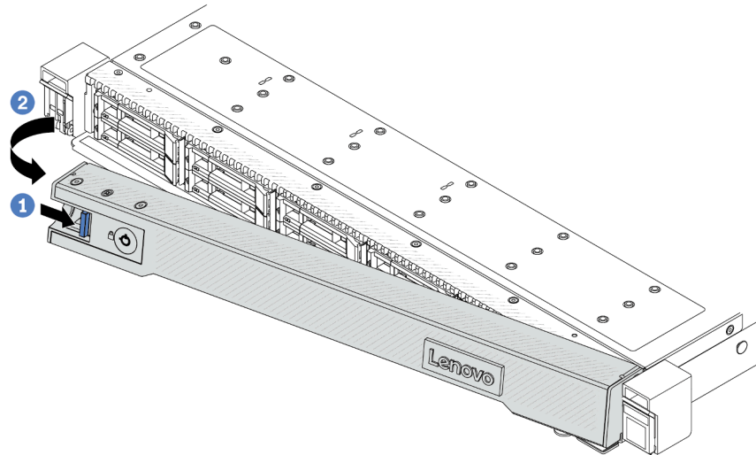
Figura 167. Extracción del marco biselado de seguridad
