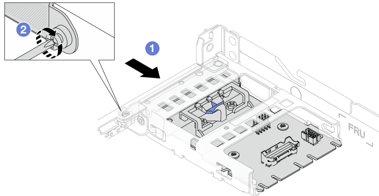
Figura 38. Instalación del intercalador OCP trasero
