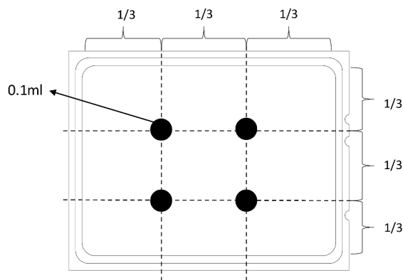
Figura 94. Aplicación de grasa térmica
