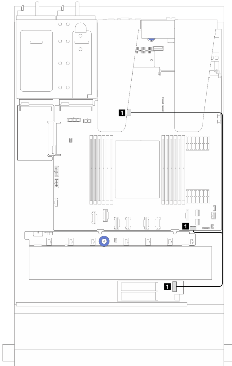
Figura 225. Disposición de los cables para ThinkSystem M.2 RAID B540i-2i SATA/NVMe Enablement Kit
