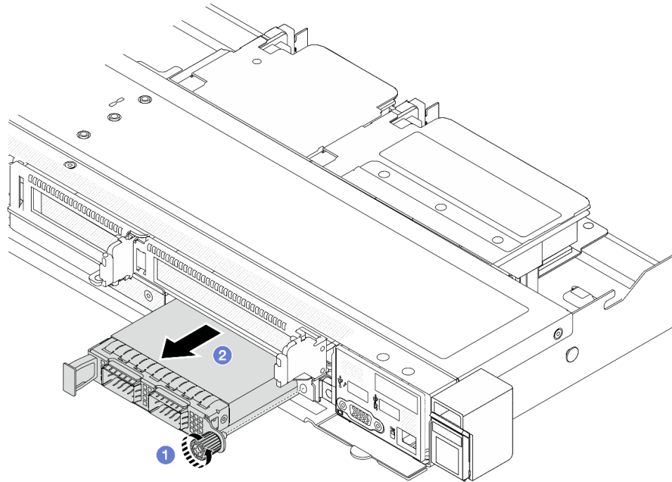
Figura 33. Extracción del módulo de OCP frontal
