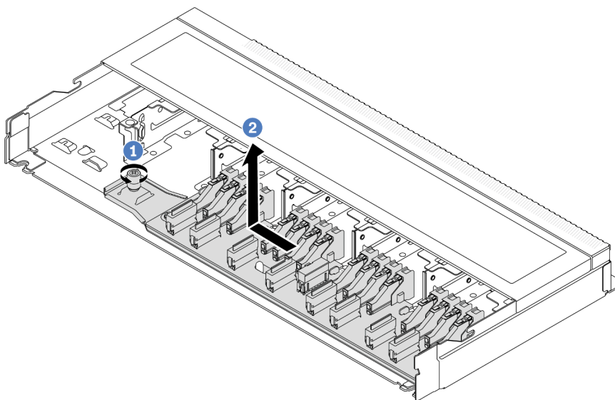
Figura 3. Extracción de la placa posterior para unidades 16 EDSFF
