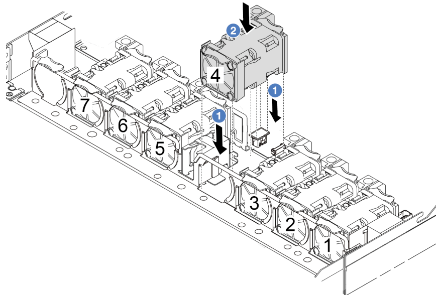
Figura 186. Instalación del ventilador del sistema
