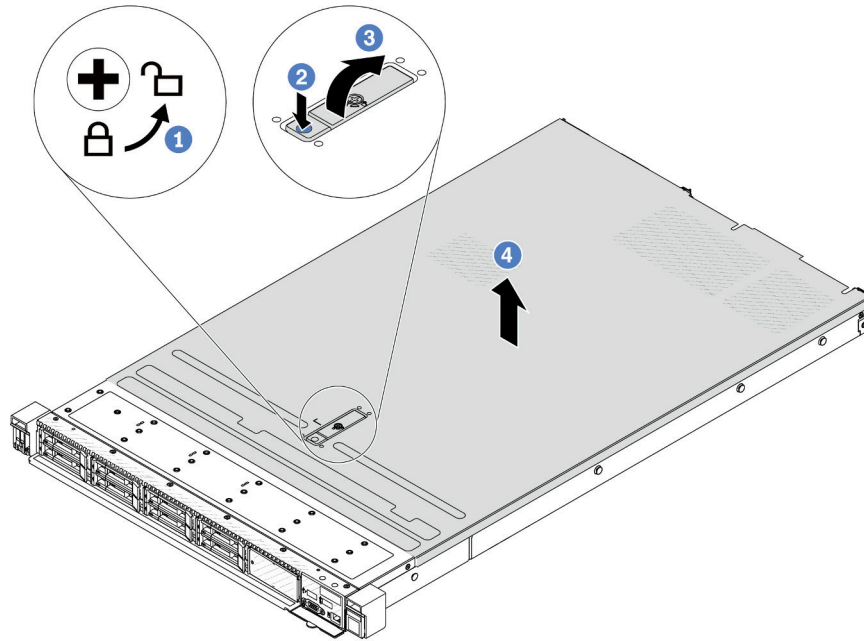
Figura 187. Extracción de la cubierta superior
