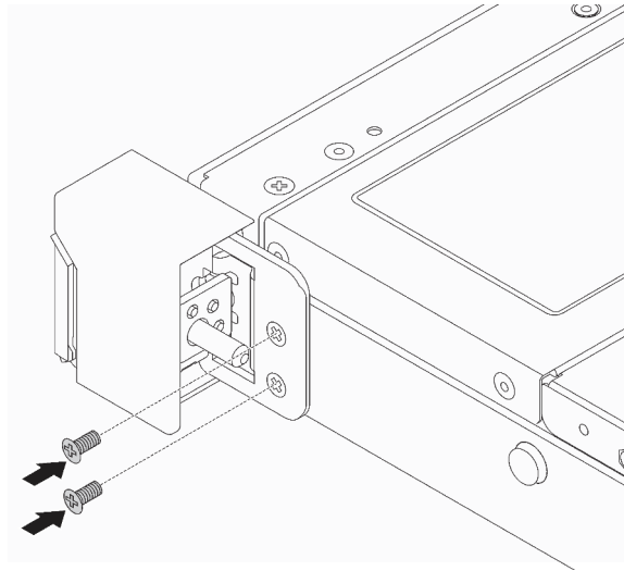
Figura 102. Instalación de tornillos del pestillo del bastidor
