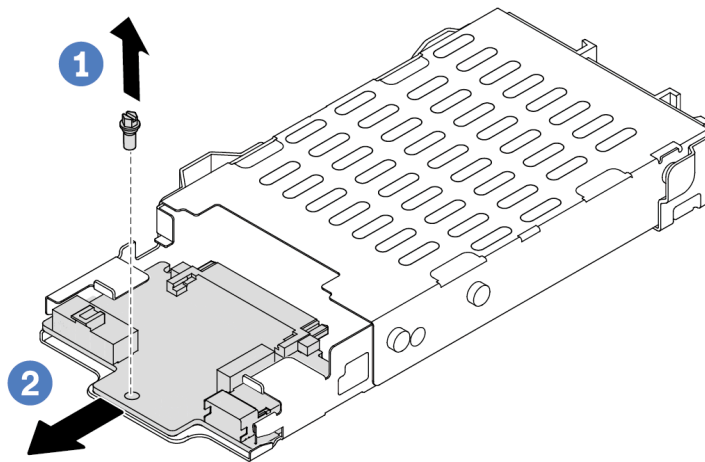
Figura 10. Extracción de la placa posterior de la unidad de 7 mm (inferior)
