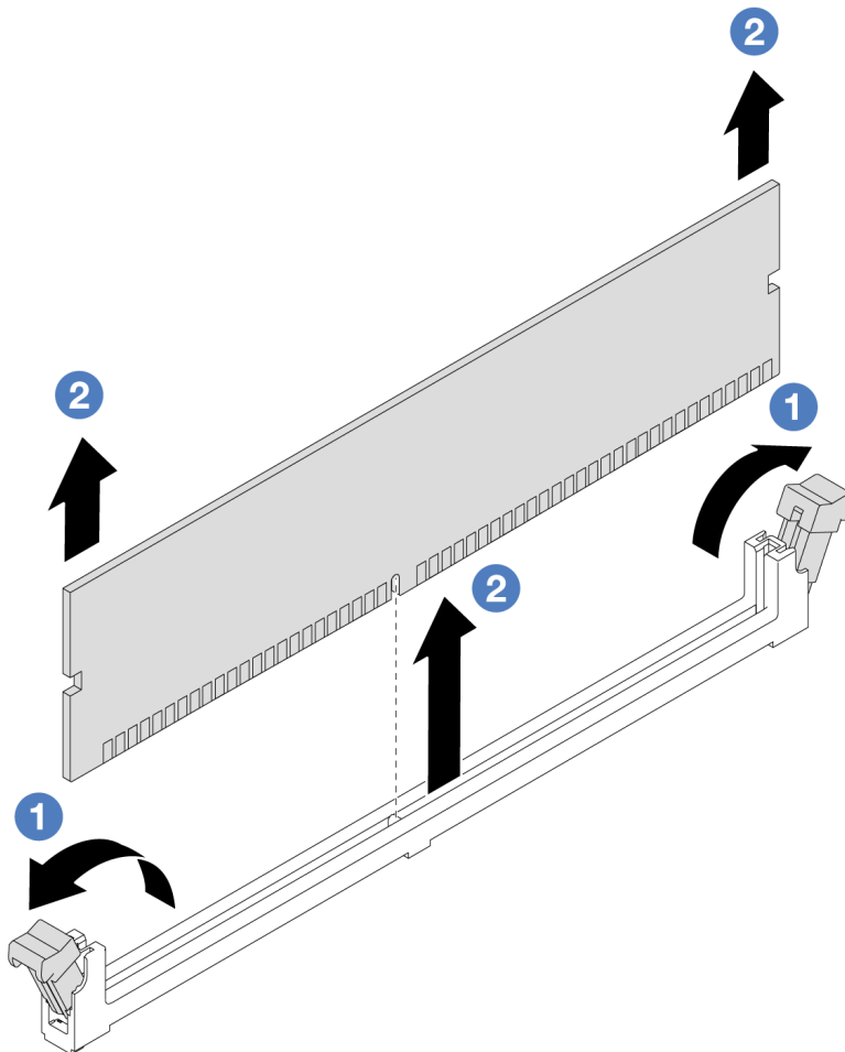
Figura 77. Extracción del módulo de memoria
