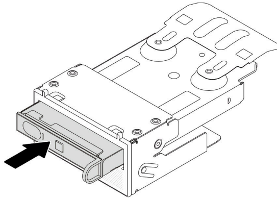
Figura 43. Instalación del panel de diagnóstico integrado en su conjunto
