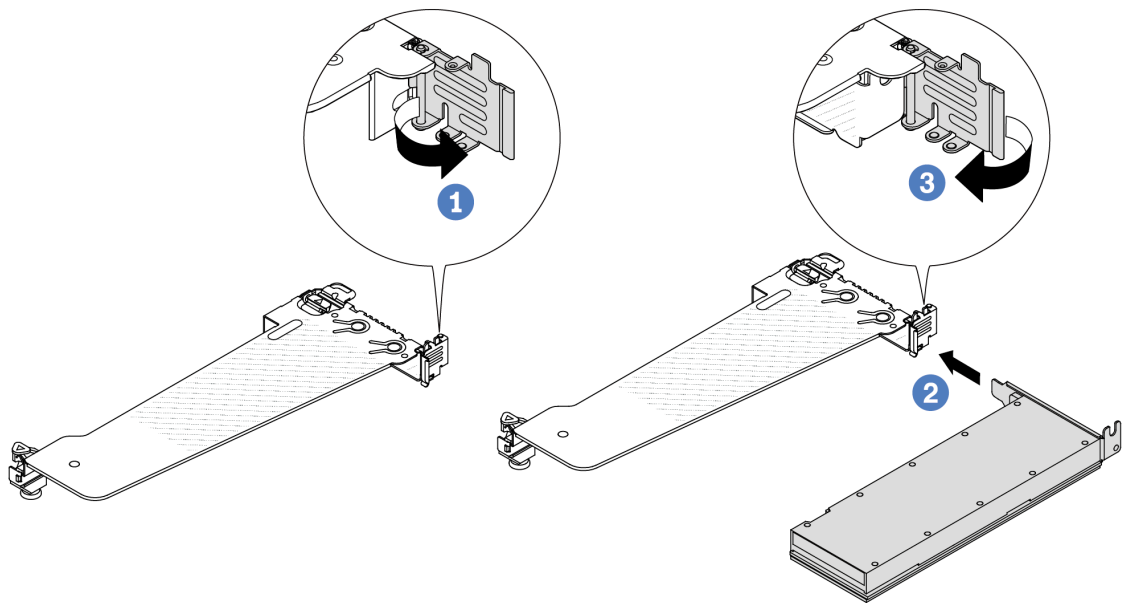
Figura 49. Instalación del adaptador GPU
