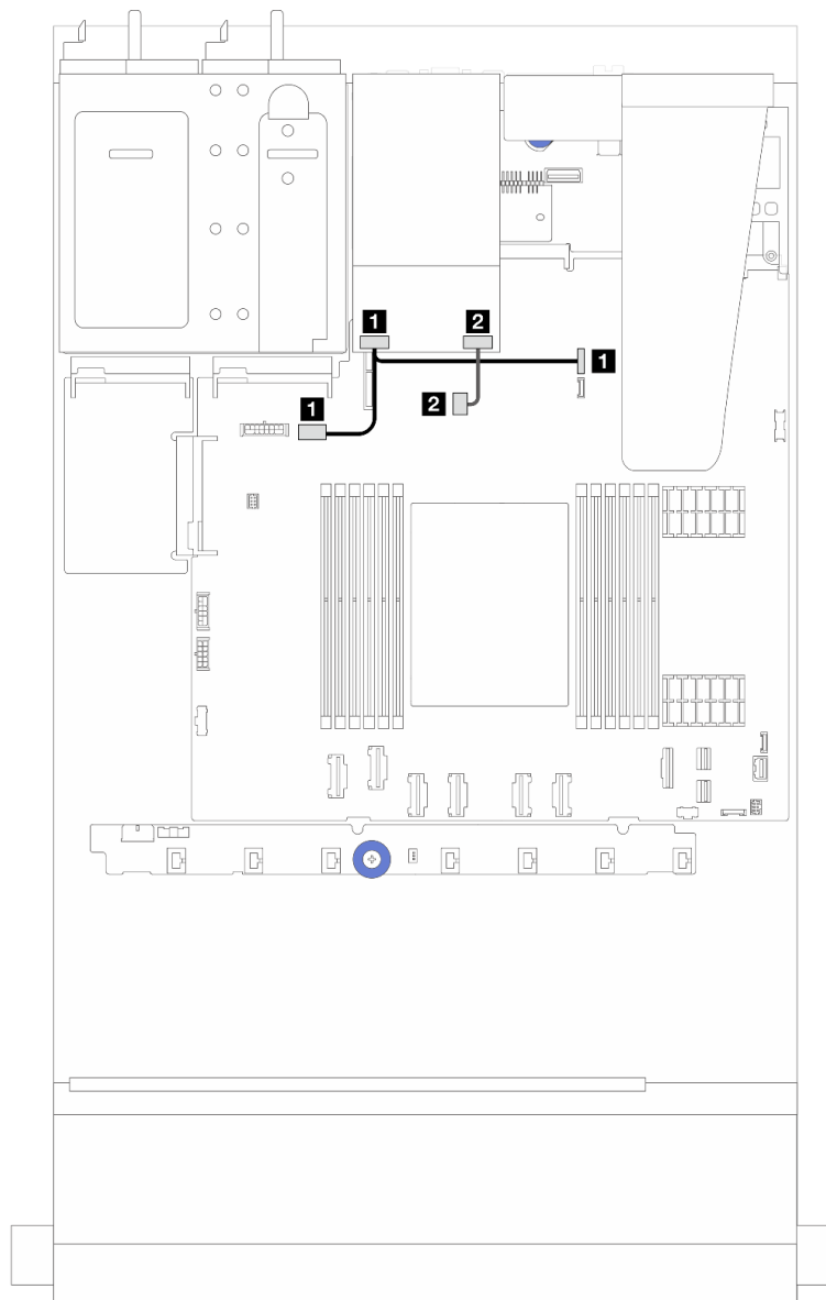
Figura 218. Disposición de los cables para placas posteriores de 7 mm de 2 bahías RAID SATA/NVMe
