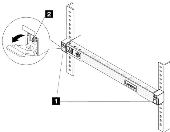
Figura 51. Desenganche del servidor del bastidor
