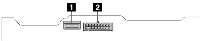
Figura 199. Placa posterior trasera de 2 unidades SAS/SATA de 2,5"
