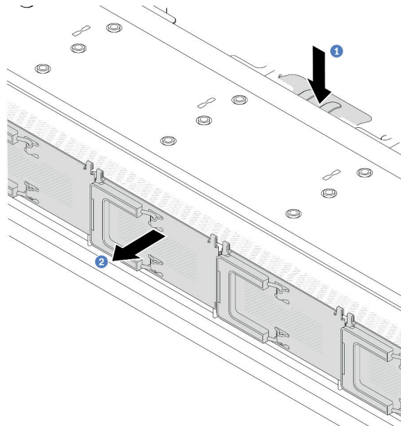
Figura 15. Extracción de compartimiento EDSFF
