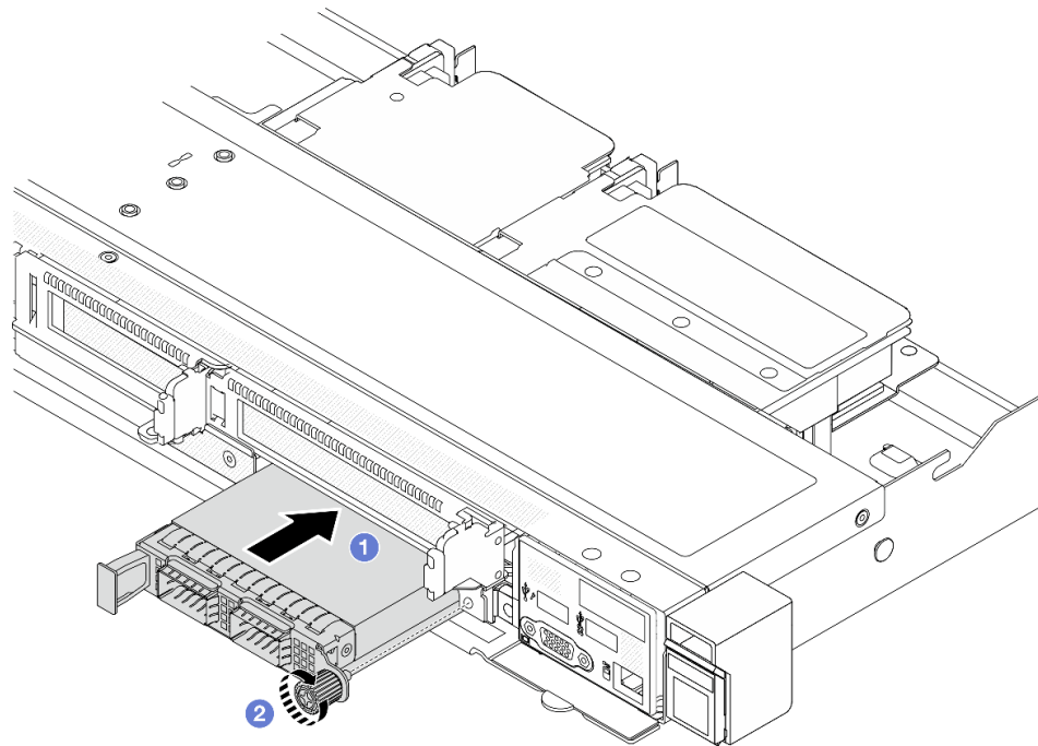
Figura 34. Instalación del módulo de OCP frontal
