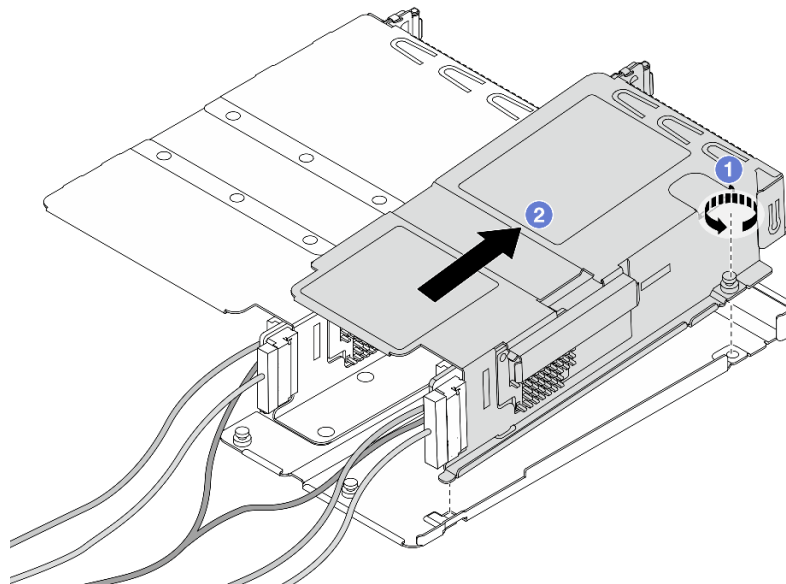
Figura 25. Separación de los dos compartimientos
