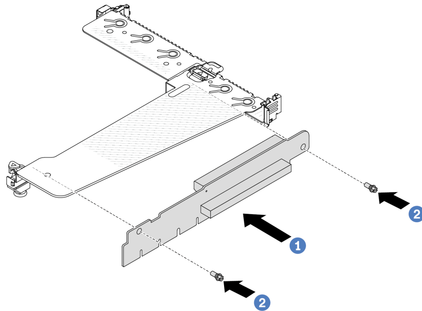
Figura 151. Instalación de la tarjeta de sujeción
