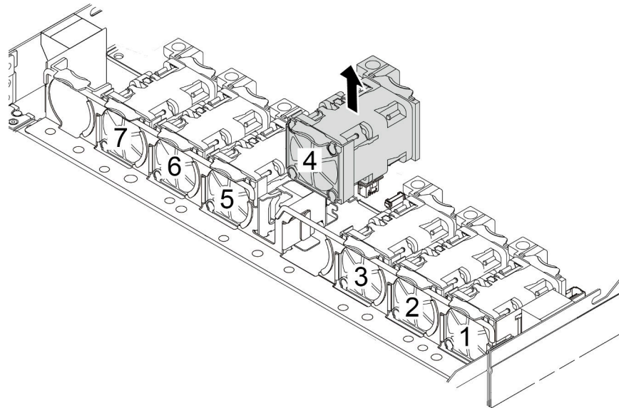
Figura 185. Extracción del ventilador del sistema
