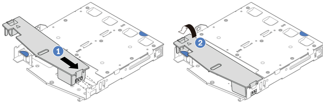
Figura 161. Instalación del deflector de aire
