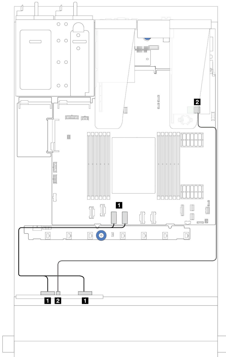
Figura 233. Disposición de los cables de 4 bahías de unidad NVMe frontales de 2,5" (con placa posterior AnyBay de 4 x 2,5" (Gen 5)) y un adaptador SFF 8i RAID/HBA (Gen 3/Gen 4)
