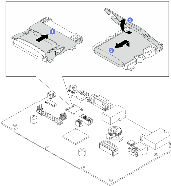
Figura 85. Extraer la tarjeta MicroSD
