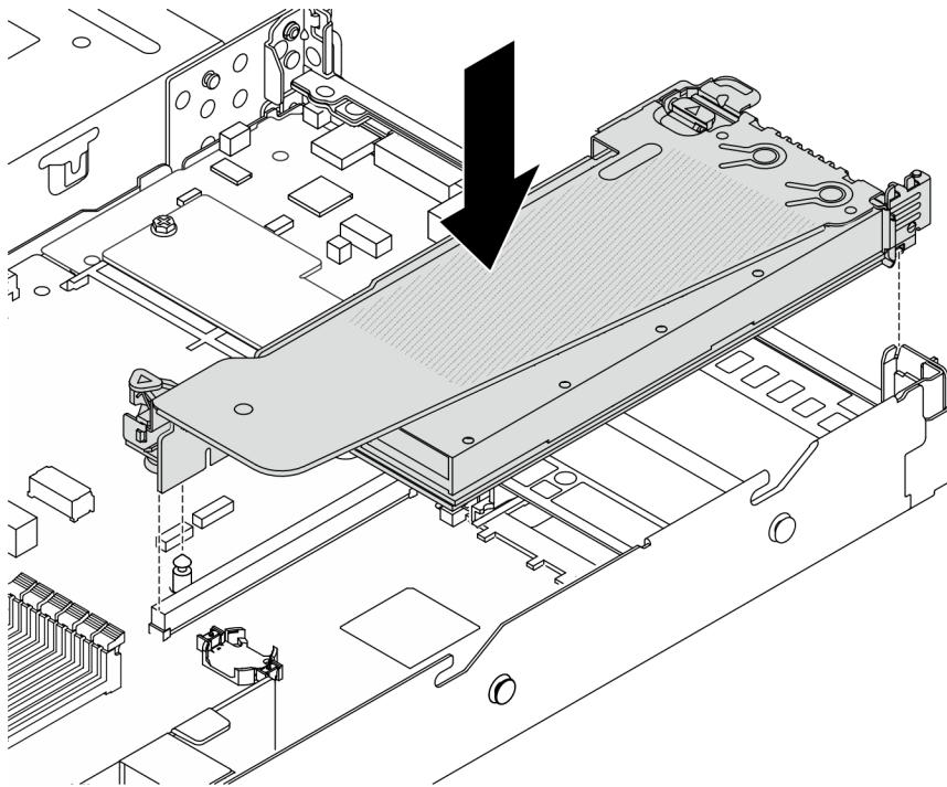
Figura 50. Instalación del conjunto de expansión
