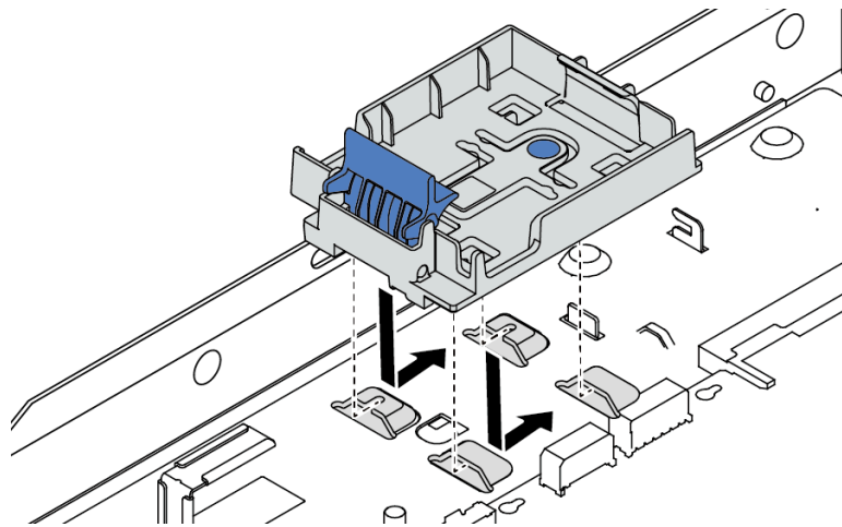
Figura 112. Instalación del compartimento del módulo de alimentación flash RAID
