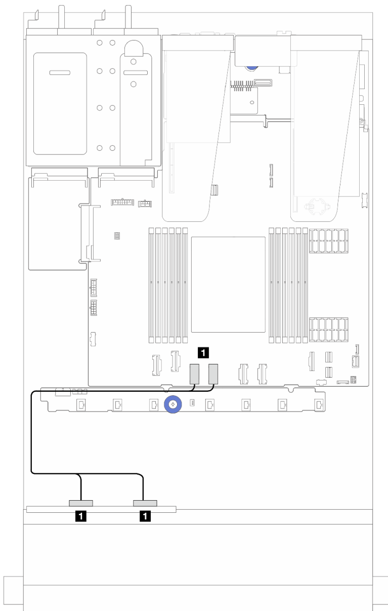
Figura 232. Disposición de los cables para la configuración integrada de 4 bahías de unidad NVMe frontales de 2,5" (con placa posterior AnyBay de 4 x 2,5" (Gen 5))
