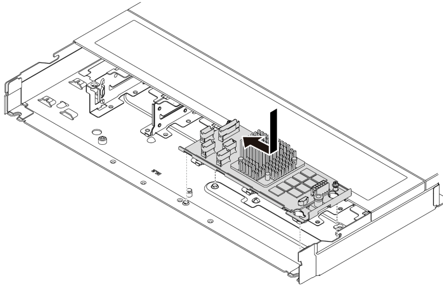
Figura 73. Instalación del adaptador HBA/RAID CFF interno
