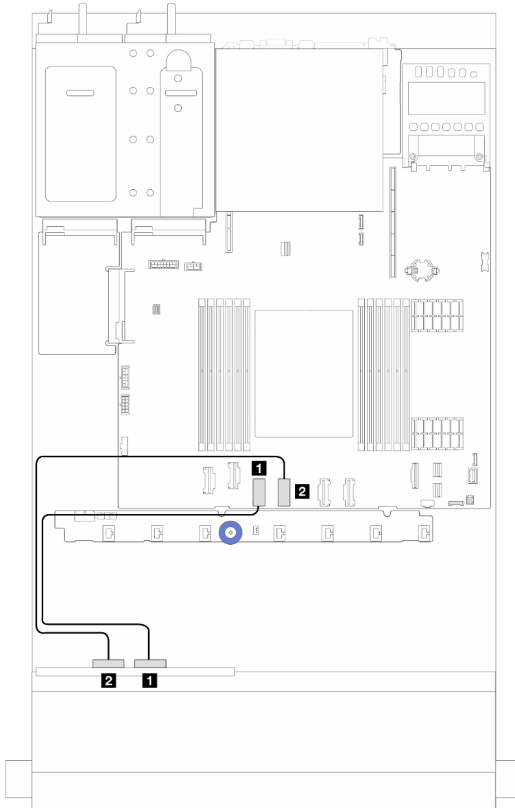
Figura 231. Disposición de los cables para la configuración integrada de 4 bahías de unidad NVMe frontales de 2,5" (con placa posterior AnyBay de 4 x 2,5" (Gen 4))
