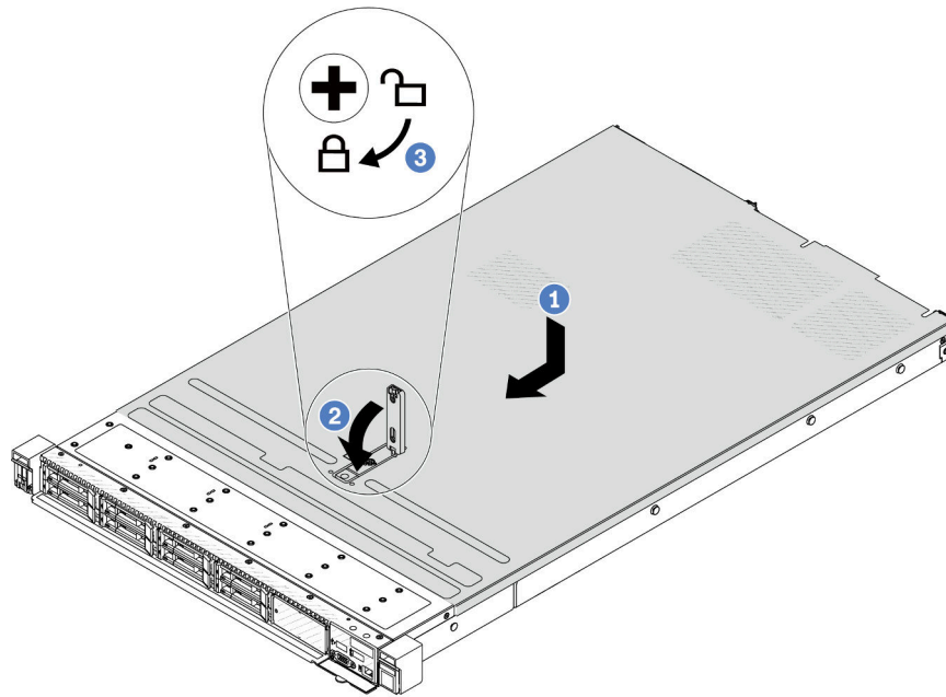
Figura 188. Instalación de la cubierta superior
