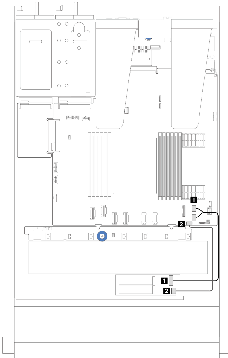
Figura 223. Disposición de los cables SATA/NVMe
