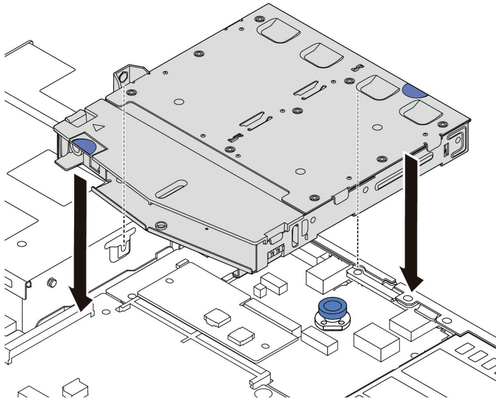
Figura 162. Instalación del compartimiento de unidad de intercambio en caliente posterior
