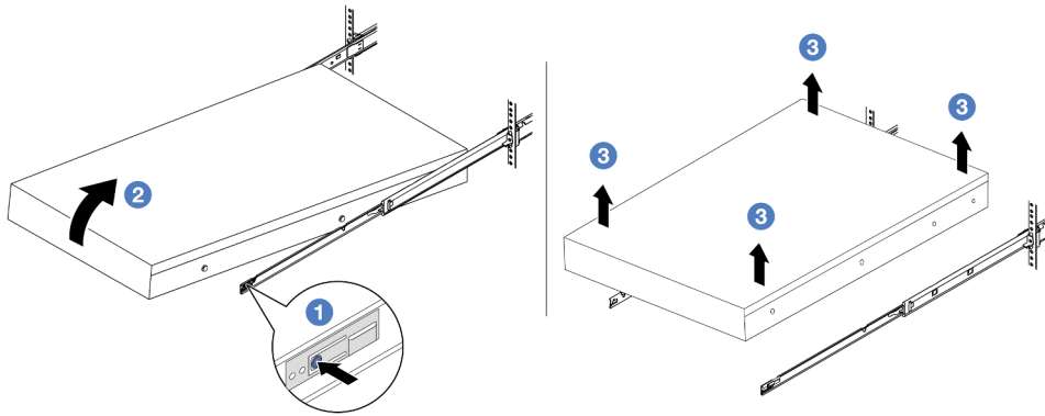
Figura 54. Extracción del servidor de un bastidor.
