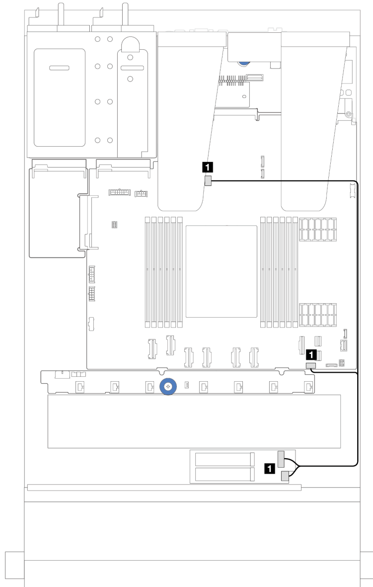
Figura 222. Disposición de los cables para ThinkSystem M.2 NVMe 2-Bay RAID Enablement Kit
