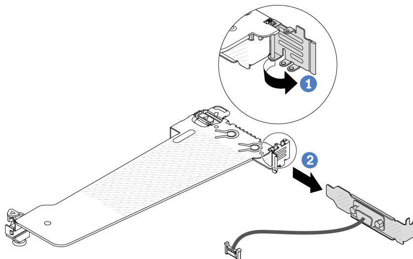
Figura 172. Extracción de la abrazadera de expansión
