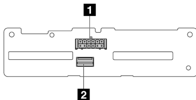
Figura 194. Placa posterior de 4 SAS/SATA de 2,5 pulgadas
