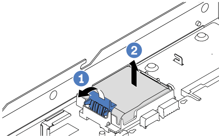
Figura 109. Extracción del módulo de alimentación flash RAID en la bandeja de la placa del sistema
