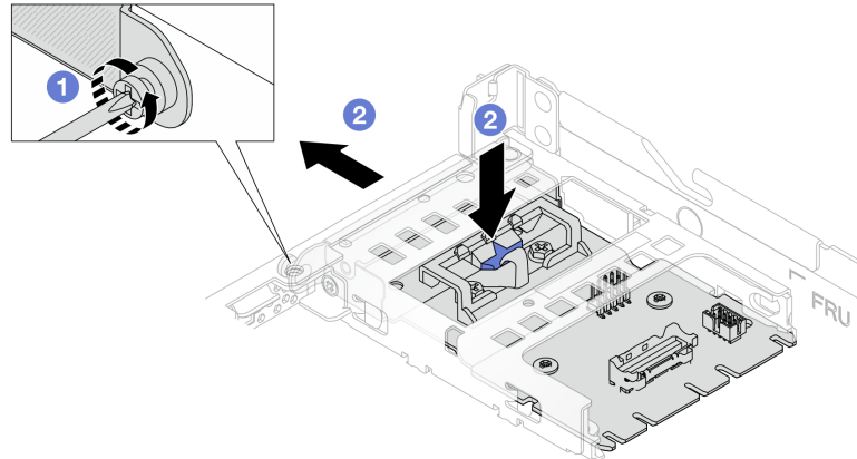
Figura 37. Extracción de la tarjeta de interposición de OCP trasera
