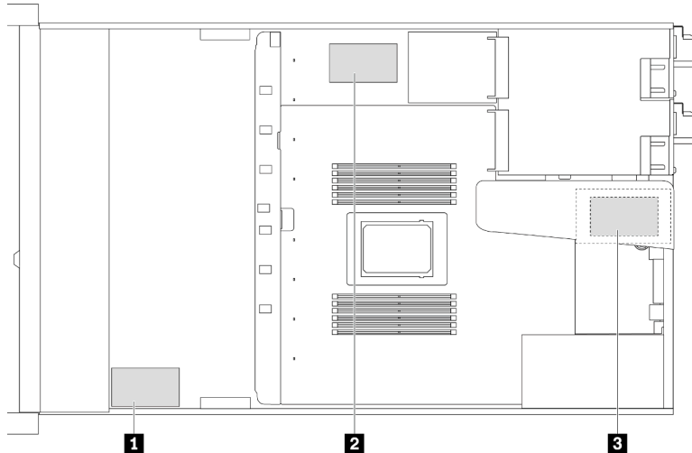
Figura 103. Módulos de alimentación flash RAID en el chasis
