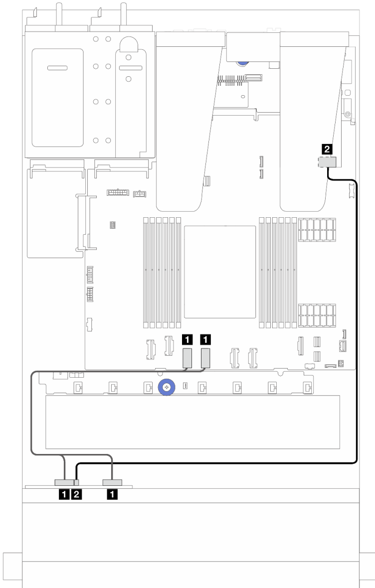
Figura 234. Disposición de los cables para 4 unidades de placa posterior AnyBay de 2,5" con un adaptador RAID SFF 8i (Gen 3 o Gen 4)
