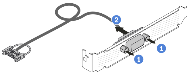
Figura 173. Desensamblaje del módulo de puerto serie
