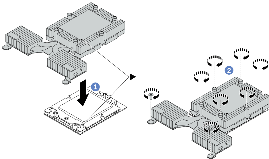
Figura 95. Instalación de un disipador de calor de refrigeración de aire
