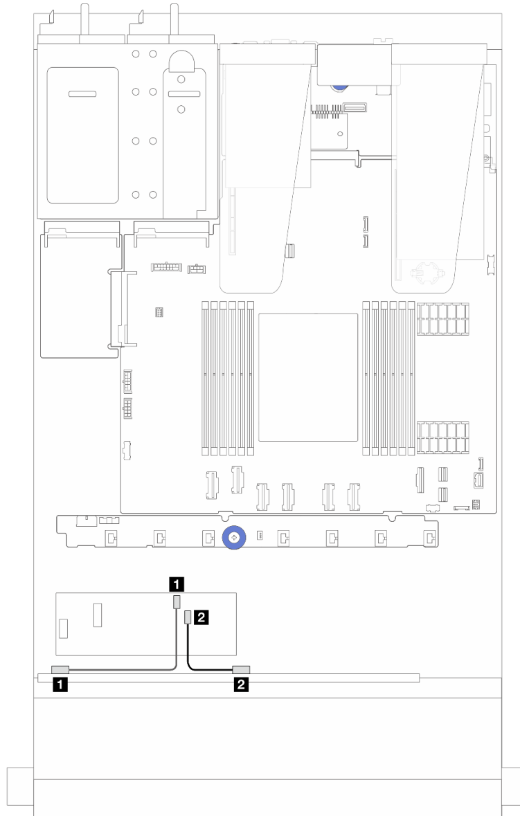
Figura 251. Disposición de los cables para 6 unidades SAS/SATA, 2 unidades AnyBay y 2 bahías de unidad NVMe frontal con un adaptador RAID CFF 8i (Gen 3)
