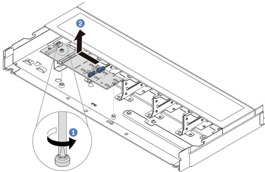
Figura 80. Extracción del módulo M.2
