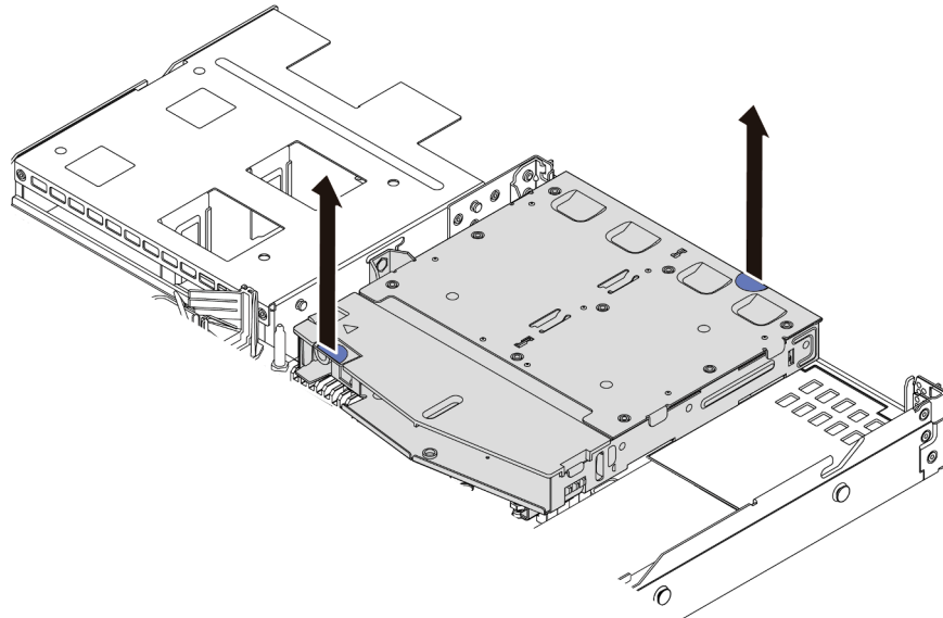
Figura 158. Extracción del compartimiento de unidad posterior de intercambio en caliente
