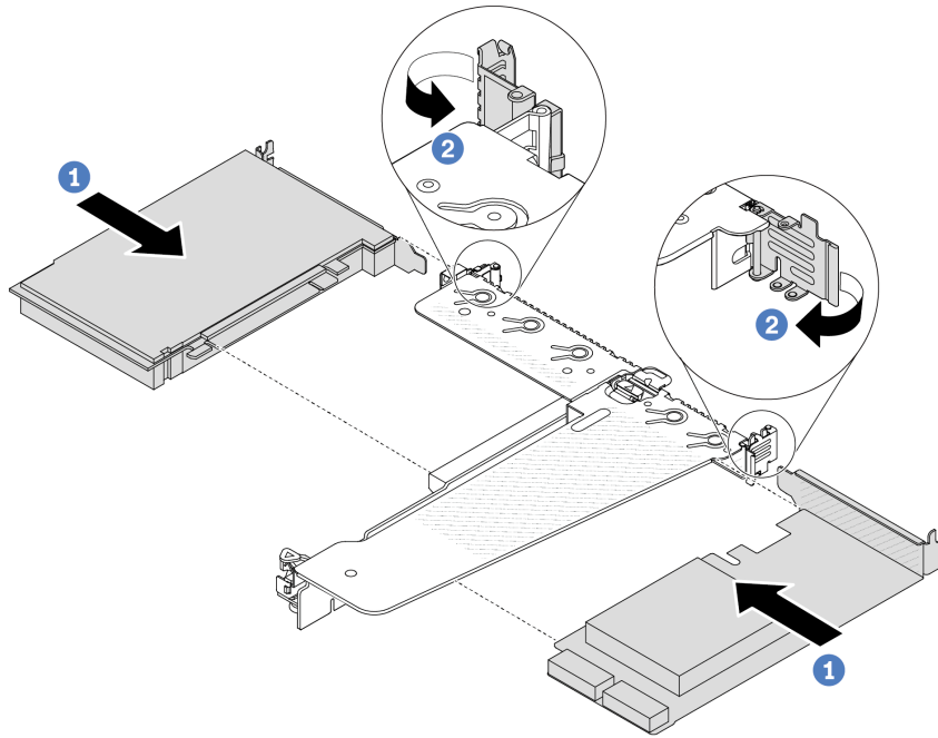
Figura 88. Instalación del adaptador PCIe en el conjunto de expansión LP-FH
