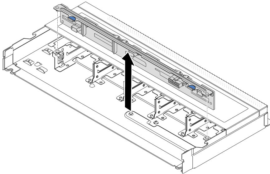
Figura 1. Extracción de la placa posterior de diez unidades de 2,5" de intercambio en caliente
