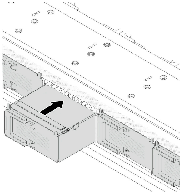
Figura 16. Instalación de compartimiento EDSFF
