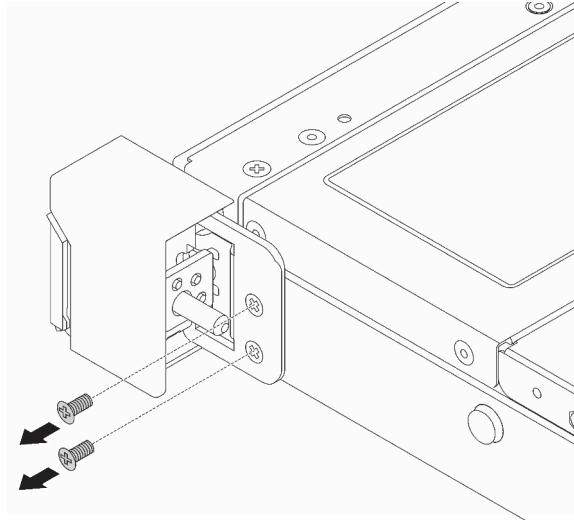
Figura 99. Extracción de los tornillos del pestillo del bastidor
