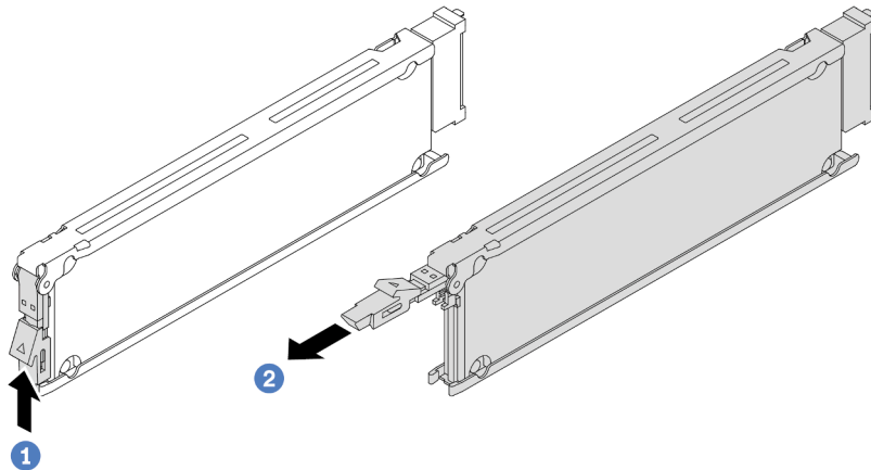
Figura 63. Extracción de la unidad EDSFF
