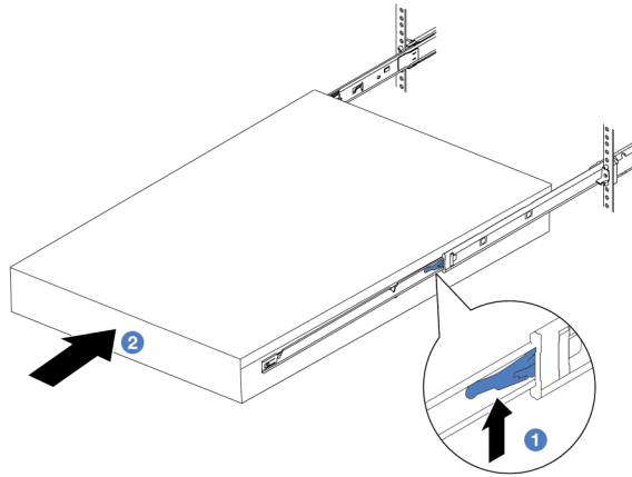
Figura 57. Instalación del servidor en el bastidor
