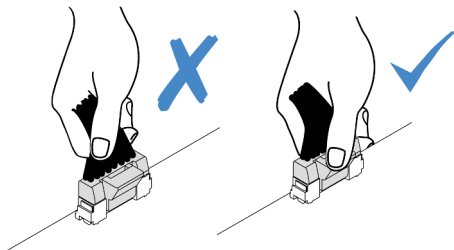
Figura 163. Desconexión de los cables del conjunto de la placa del sistema
