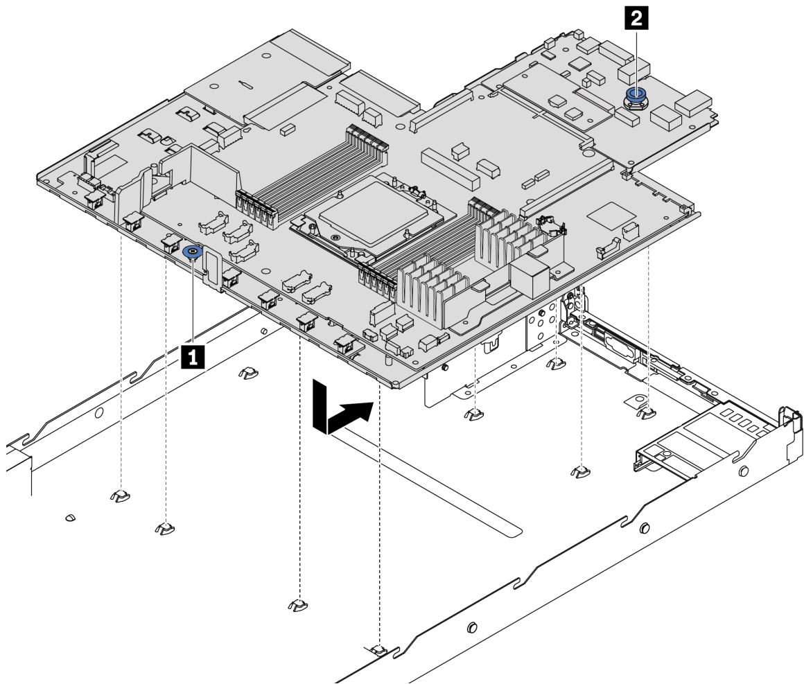
Figura 184. Instalación del conjunto de la placa del sistema
