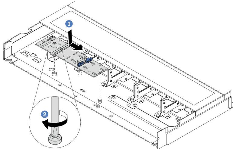
Figura 83. Instalación de la placa posterior de M.2
