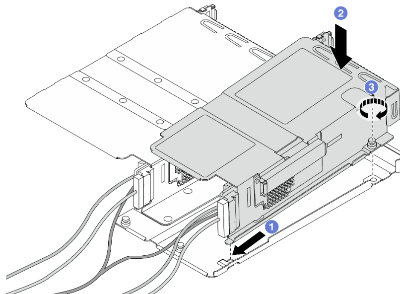
Figura 32. Montaje de los dos compartimentos de expansión
