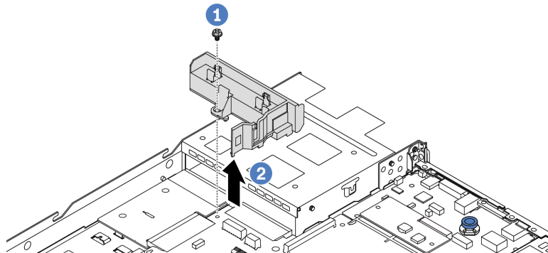
Figura 89. Extracción del deflector de aire de la unidad de fuente de alimentación
