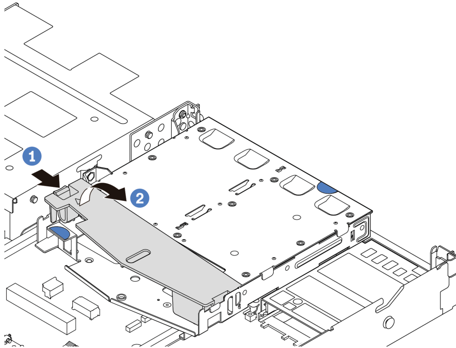
Figura 159. Extracción del deflector de aire
