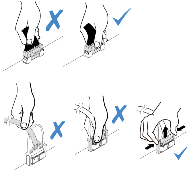
Figura 180. Desconexión de los cables del conjunto de la placa del sistema
