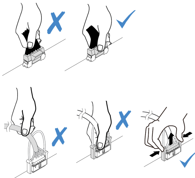
Figura 39. Desconexión de los cables del conjunto de la placa del sistema
