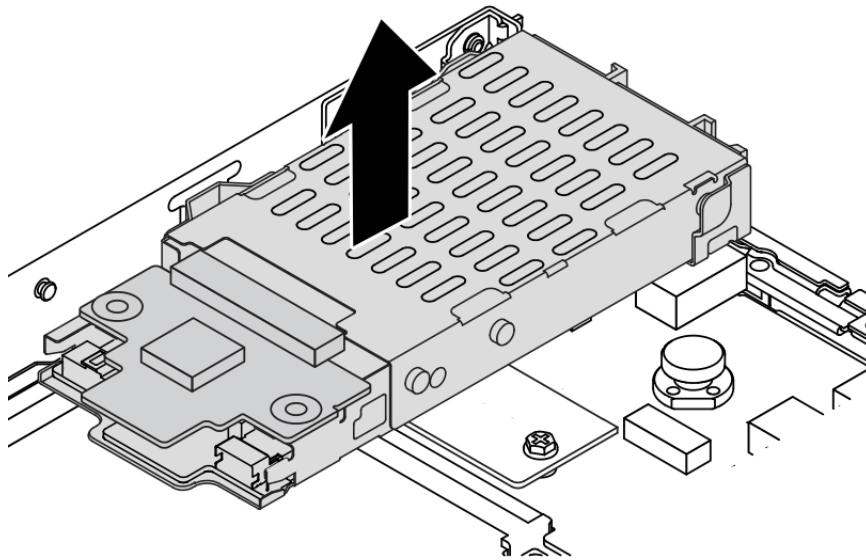
Figura 164. Extracción del compartimiento de unidad posterior de intercambio en caliente
