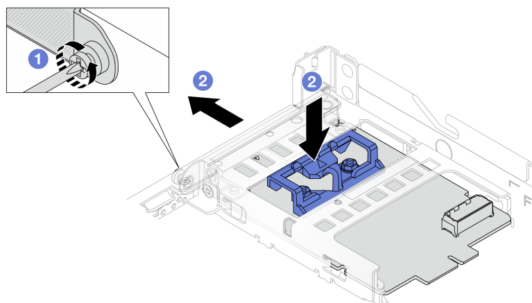
Figura 75. Extracción del adaptador NIC de gestión
