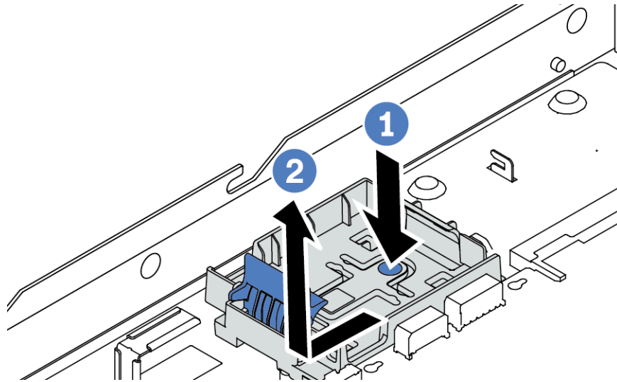
Figura 110. Extracción del compartimento del módulo de alimentación flash RAID
