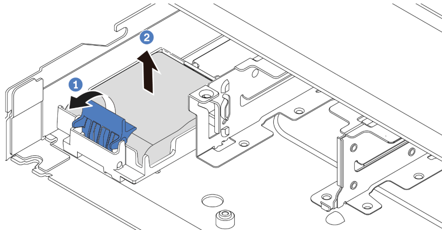
Figura 104. Extracción del módulo de alimentación flash RAID en el chasis
