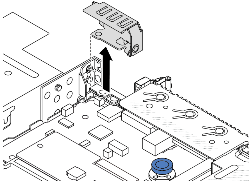
Figura 150. Extracción de la abrazadera de pared posterior
