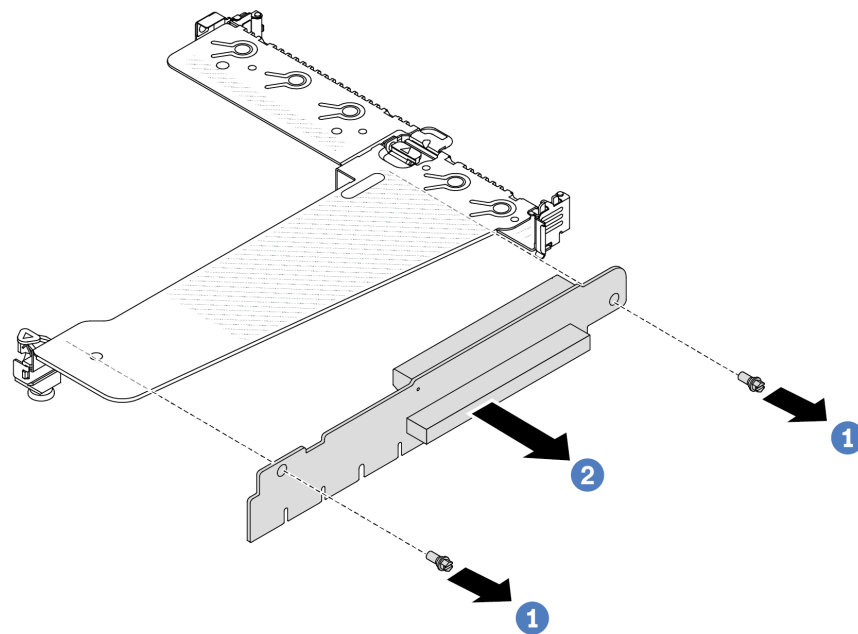
Figura 149. Extracción de la tarjeta de expansión
