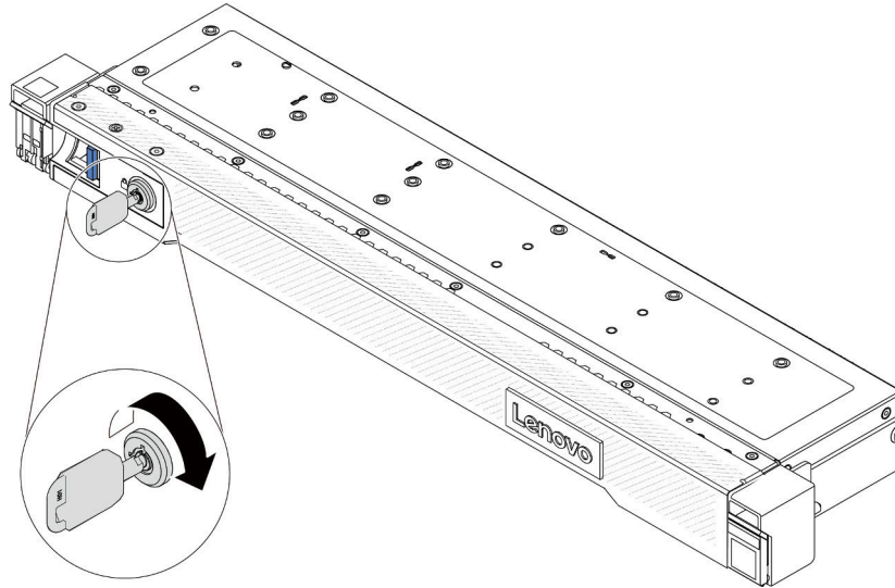
Figura 166. Desbloqueo del marco biselado de seguridad
