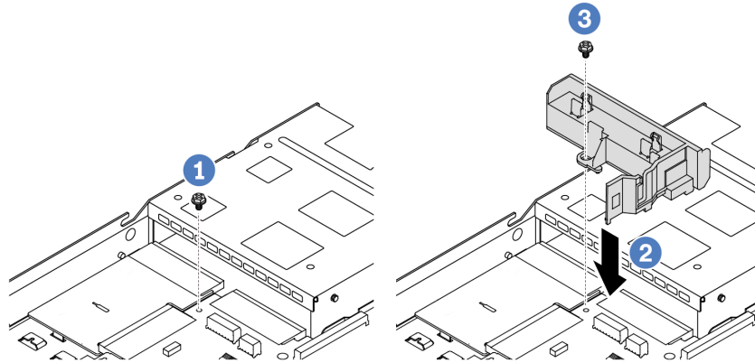
Figura 90. Instalación del deflector de aire de la unidad de fuente de alimentación
