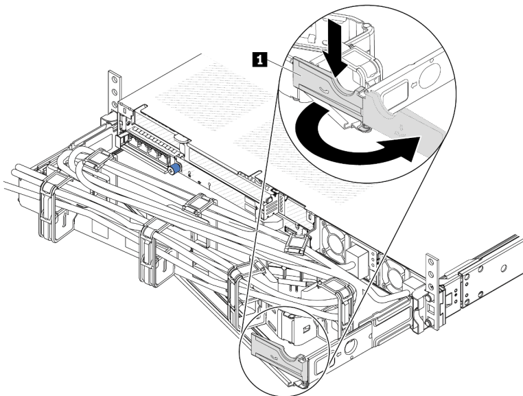
Figura 67. Ajuste la CMA
