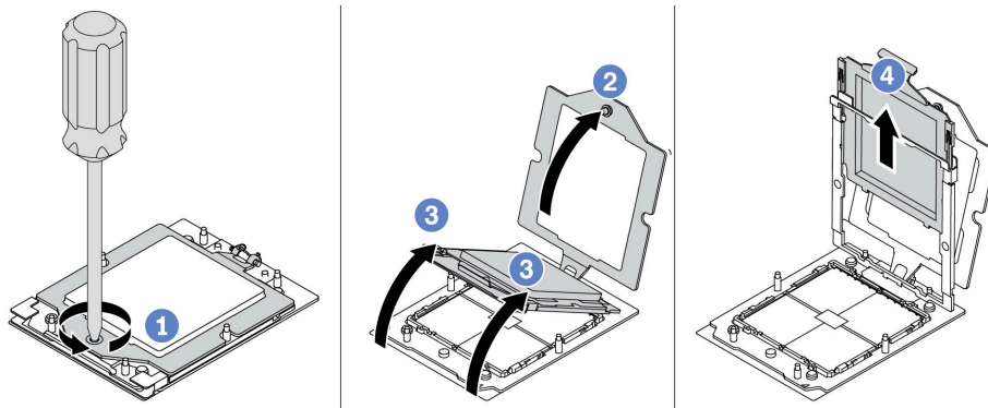
Figura 93. Extracción de un procesador
