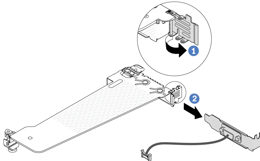
Figure 172. Retrait du support de carte mezzanine
