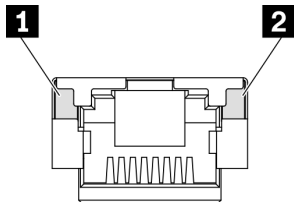
Figure 260. Voyants du Port de gestion du système XCC
