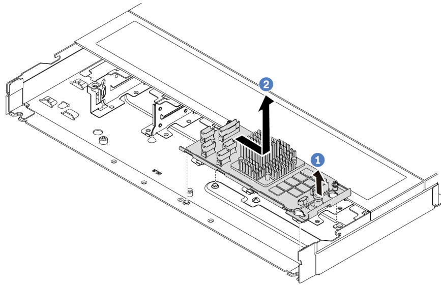
Figure 72. Retrait de l'adaptateur RAID/HBA CFF interne
