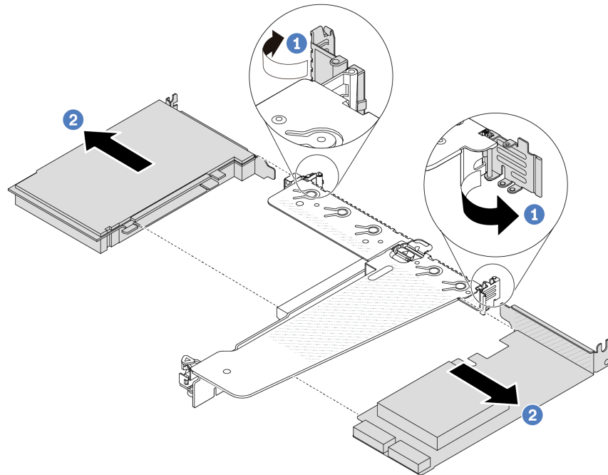
Figure 87. Retrait d'un adaptateur PCIe de l'assemblage de cartes mezzanines LP-FH
