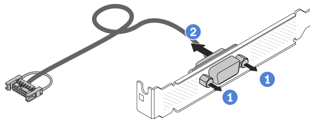
Figure 173. Démontage du module de port série
