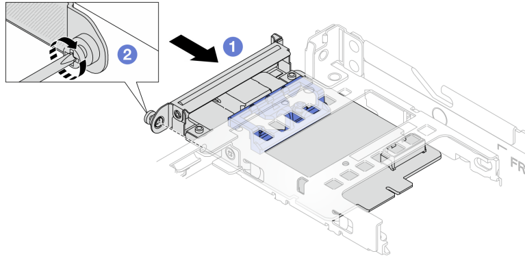
Figure 76. Installation de l'adaptateur NIC de gestion
