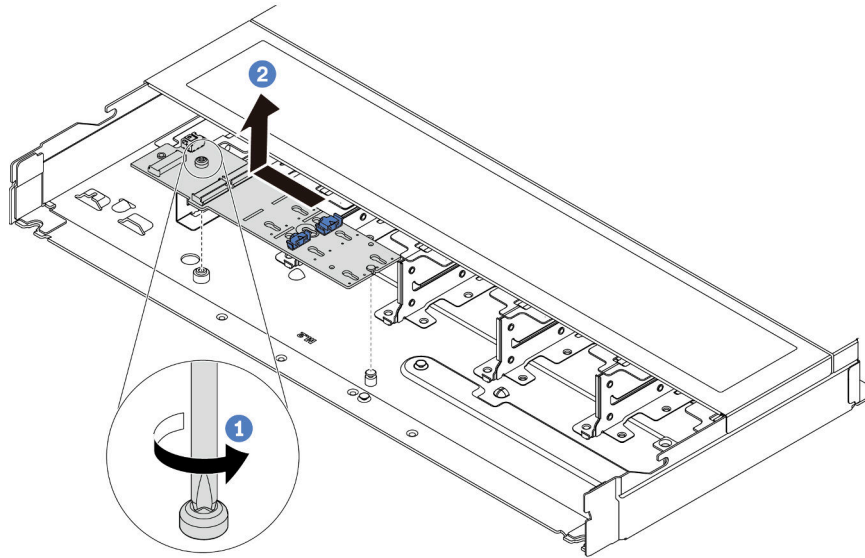
Figure 80. Retrait du module M.2
