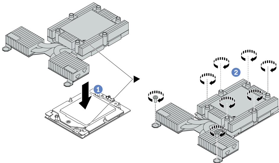
Figure 95. Installation d'un dissipateur thermique à refroidissement par air
