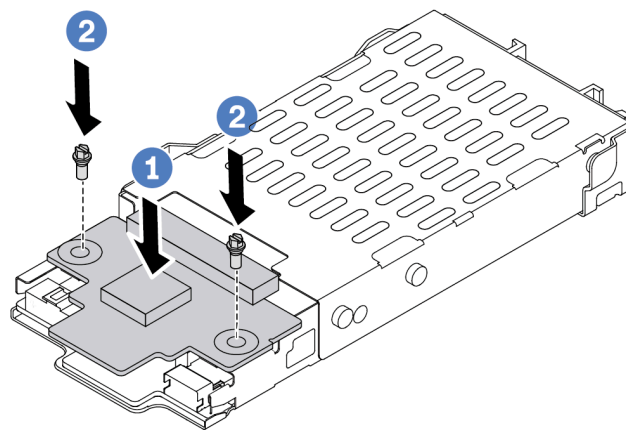
Figure 12. Installation d'un fond de panier d'unité 7 mm (haut)
