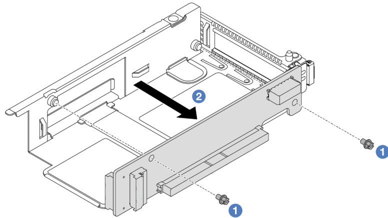
Figure 27. Retrait de la carte mezzanine du boîtier extra-plat
