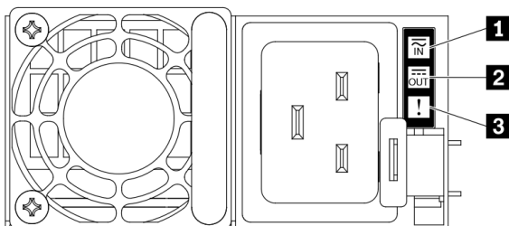
Figure 258. Voyants de l'alimentation
