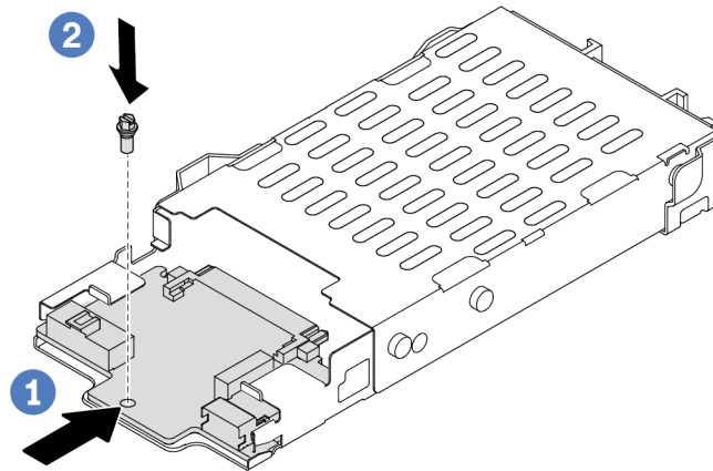
Figure 11. Installation du fond de panier d'unité 7 mm (bas)
