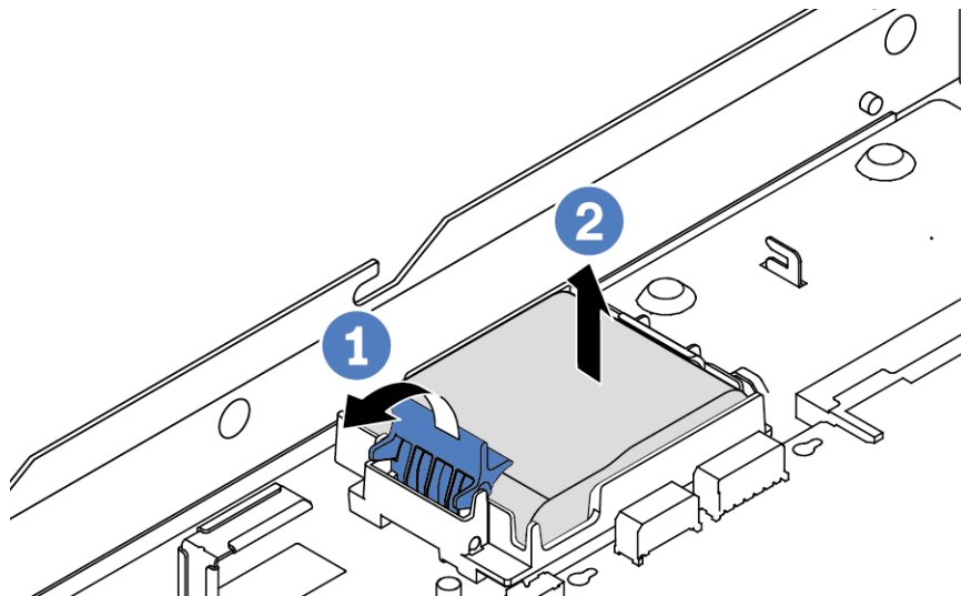
Figure 109. Retrait du module d'alimentation flash RAID du plateau de la carte mère
