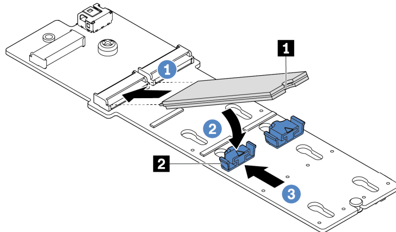
Figure 84. Installation d'une unité M.2
