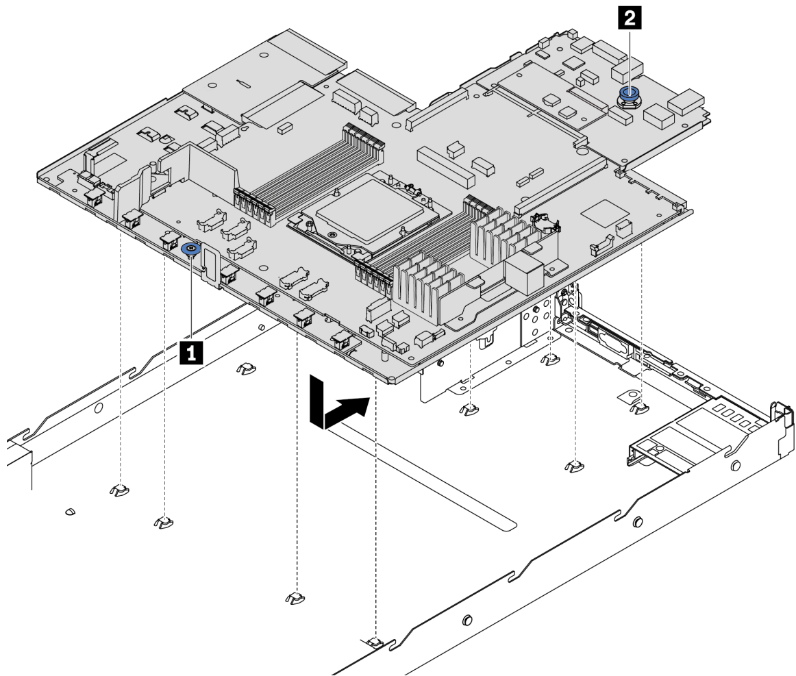
Figure 184. Installation du bloc carte mère
