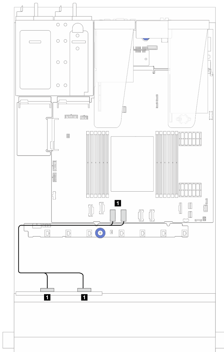
Figure 232. Cheminement des câbles pour la configuration intégrée avec des baies d'unité NVMe 4 x 2,5pouces avant (fond de panier AnyBay 4 x 2,5 pouces Gen 5)
