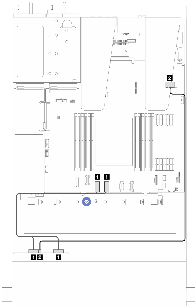
Figure 234. Cheminement des câbles pour les unités du fond de panier AnyBay 4 x 2,5 pouces avec un adaptateur RAID 8i SDD (Gen 3 ou Gen 4)
