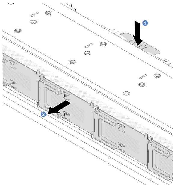
Figure 15. Retrait du boîtier d'unités EDSFF
