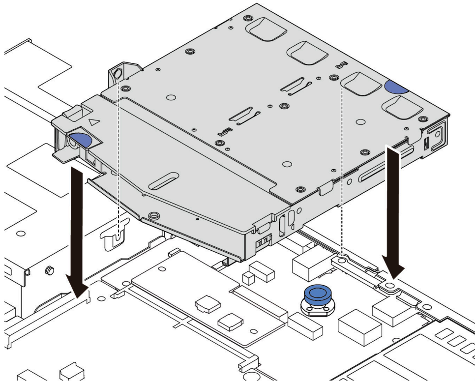
Figure 162. Installation du boîtier d'unité remplaçable à chaud arrière
