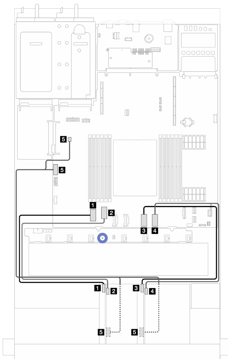
Figure 203. Cheminement des câbles de l'assemblage de cartes mezzanines avant
