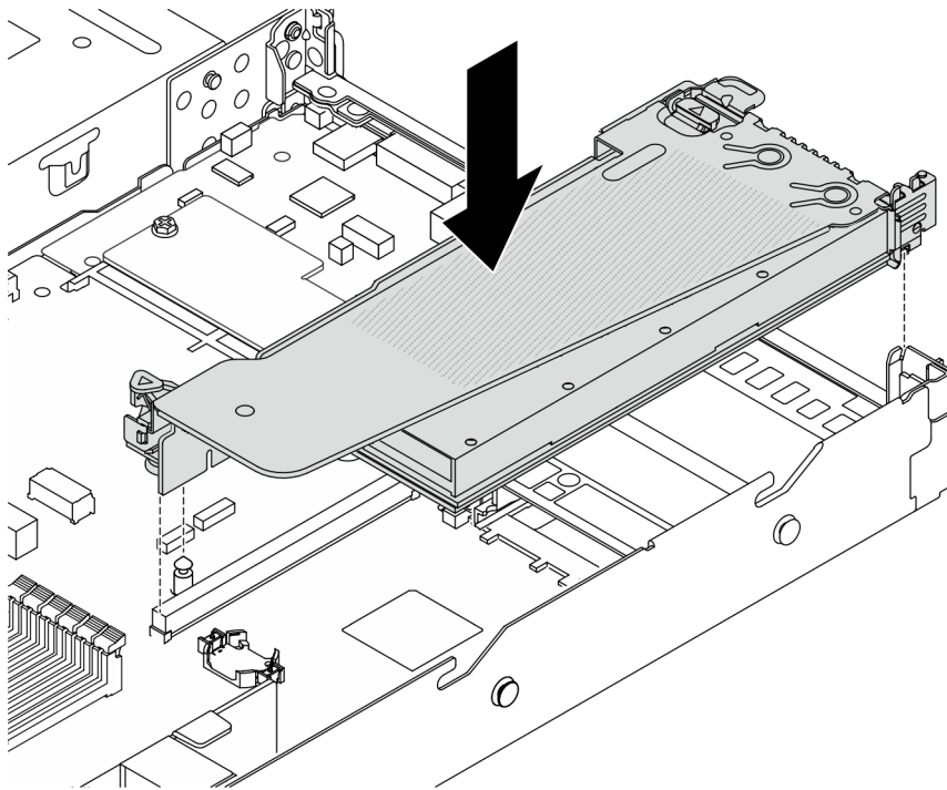
Figure 50. Installation de l'assemblage de cartes mezzanines
