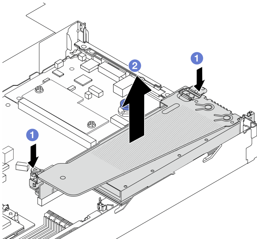
Figure 47. Retrait de l'assemblage de cartes mezzanines
