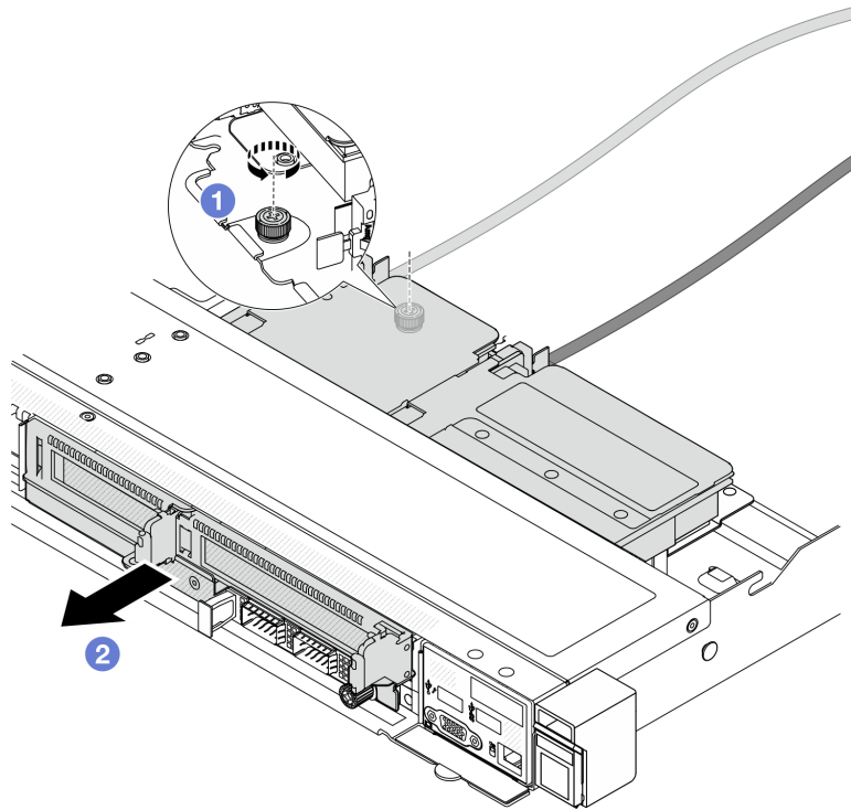
Figure 23. Retrait du boîtier de la carte mezzanine avant
