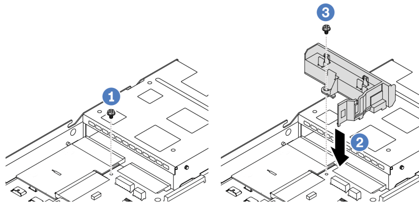
Figure 90. Installation d'une grille d'aération sur le bloc d'alimentation
