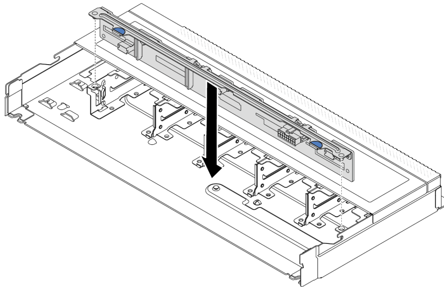
Figure 2. Installation du fond de panier pour dix unités remplaçables à chaud 2,5 pouces
