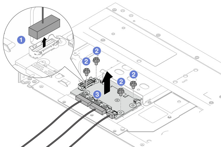
Figure 35. Retrait de la carte d'interposeur OCP avant
