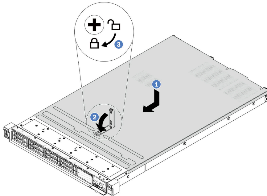
Figure 188. Installation du carter supérieur
