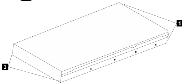
Figure 56. Levage du serveur
