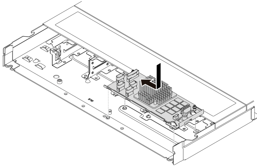
Figure 73. Installation de l'adaptateur RAID/HBA CFF interne
