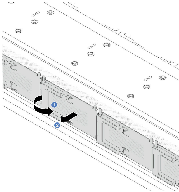
Figure 17. Retrait du couvercle du boîtier d'unités de disque dur EDSFF
