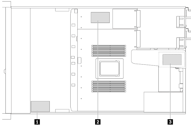
Figure 206. Modules d'alimentation flash RAID sur le châssis
