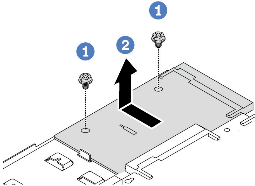
Figure 97. Retrait de la carte PIB
