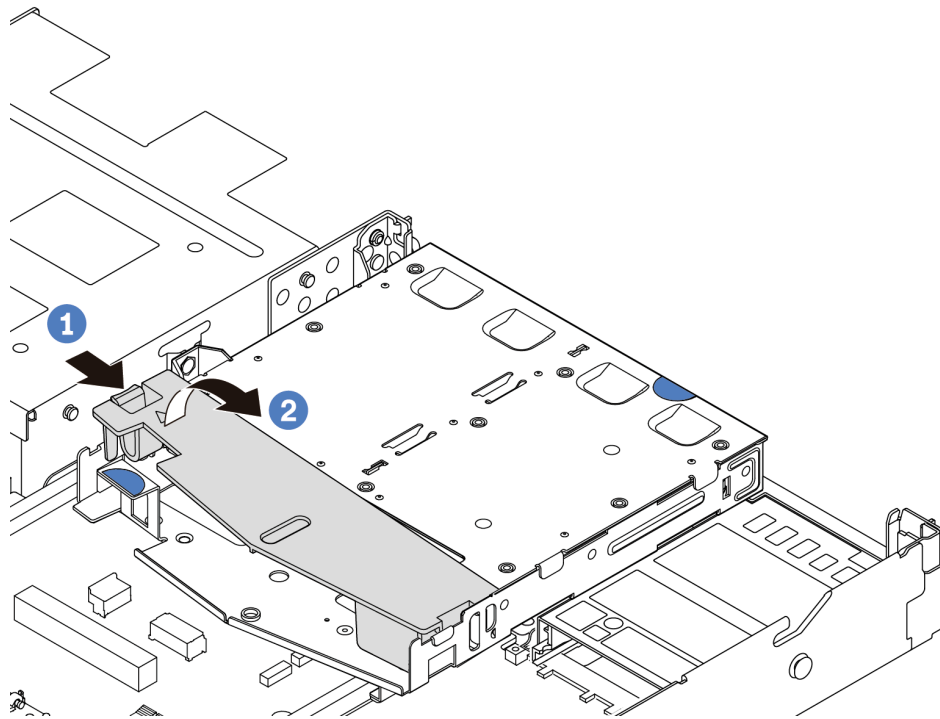
Figure 159. Retrait de la grille d'aération
