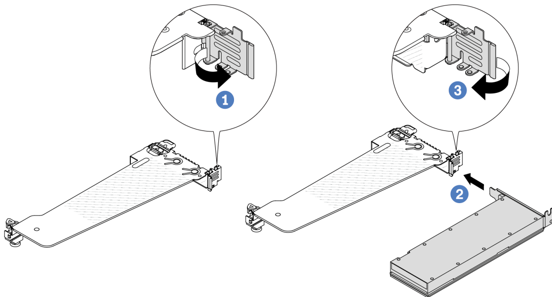
Figure 49. Installation de l'adaptateur GPU
