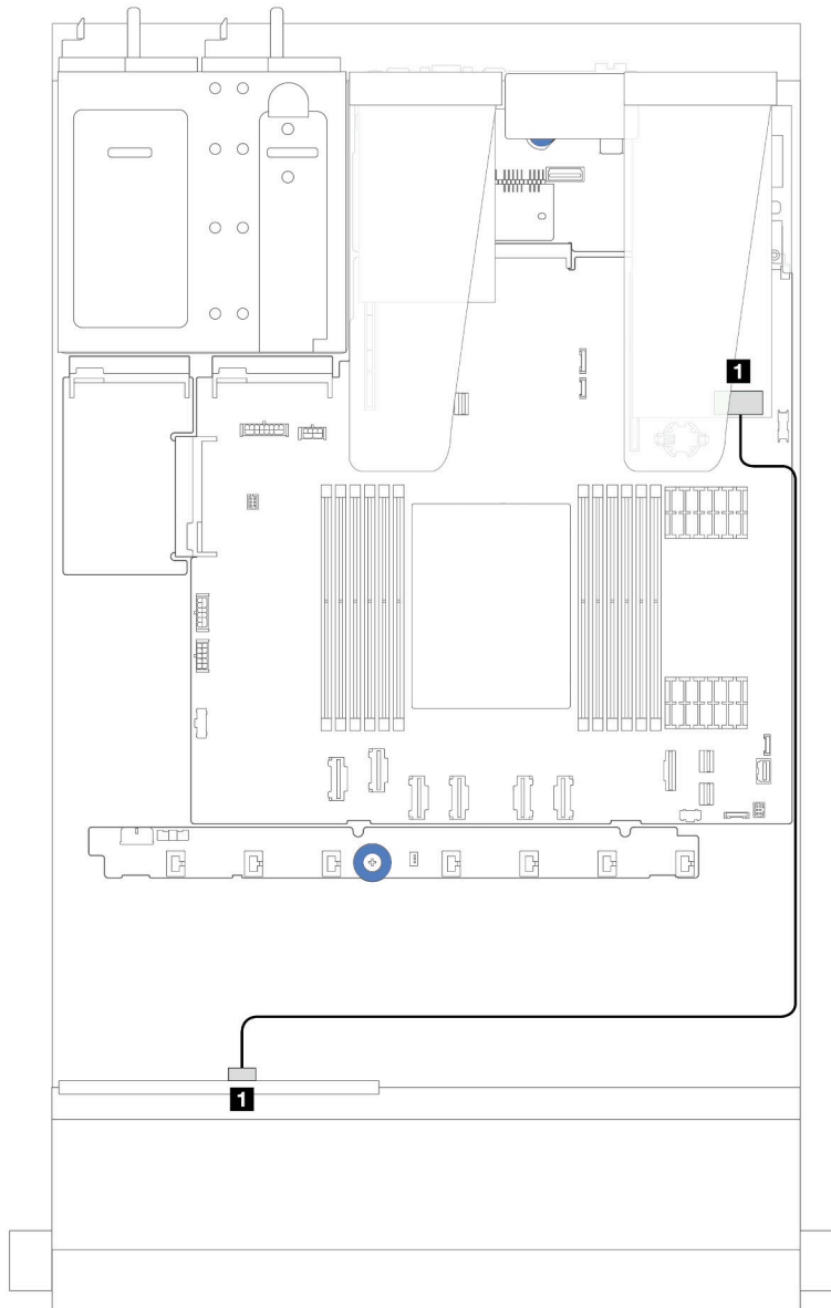
Figure 230. Cheminement des câbles pour des baies d'unité SAS/SATA 4 x 2,5 pouces avant et un adaptateur RAID 8i SFF (Gen 3/Gen 4)
