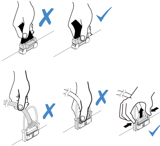
Figure 180. Déconnexion des câbles du bloc carte mère
