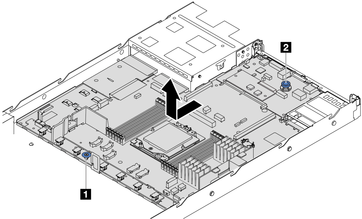
Figure 181. Retrait du bloc carte mère
