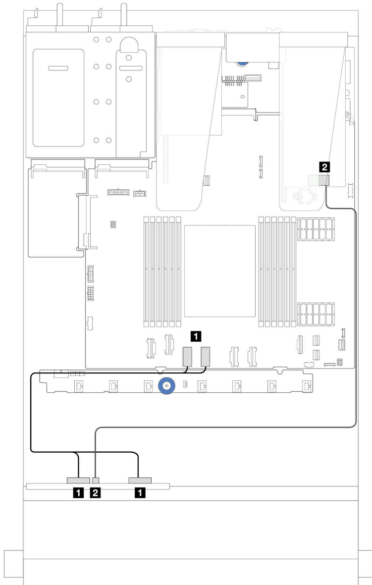
Figure 233. Cheminement des câbles des baies d'unité NVMe 4 x 2,5 pouces avant (fond de panier AnyBay 4 x 2,5 pouces Gen 5) et un adaptateur RAID/HBA 8i SFF (Gen 3/Gen 4)
