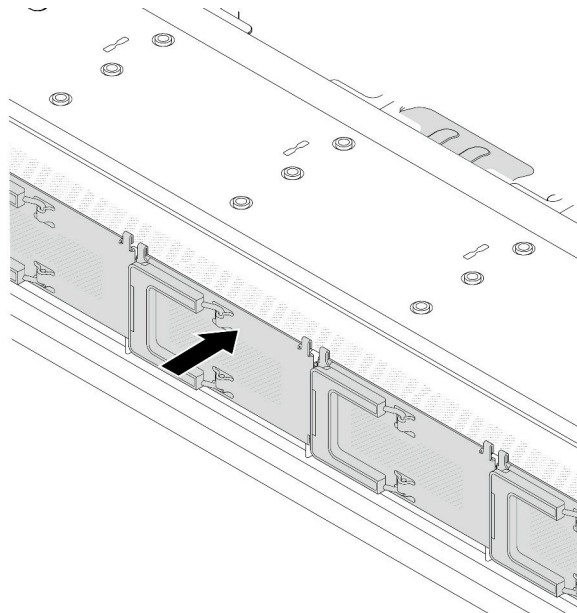
Figure 66. Installation du couvercle du boîtier d'unités de disque dur EDSFF
