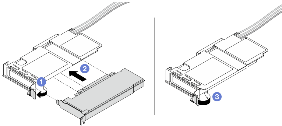
Figure 31. Installation de l'adaptateur PCIe
