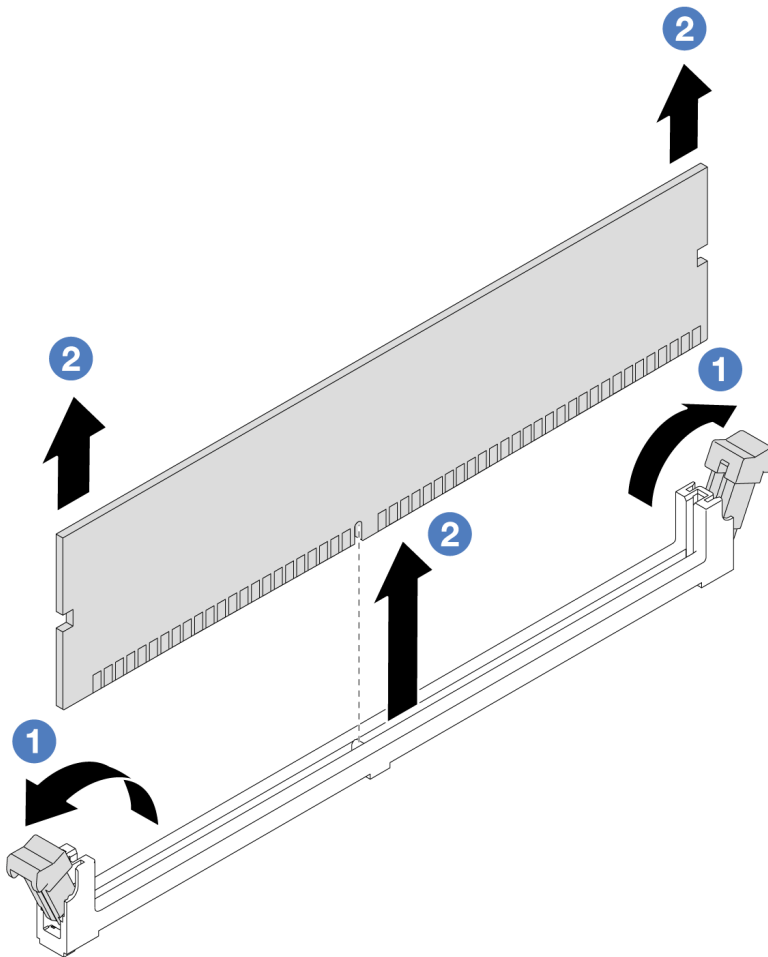
Figure 77. Retrait d'un module de mémoire
