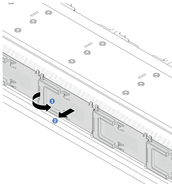
Figure 62. Retrait du couvercle du boîtier d'unités de disque dur EDSFF
