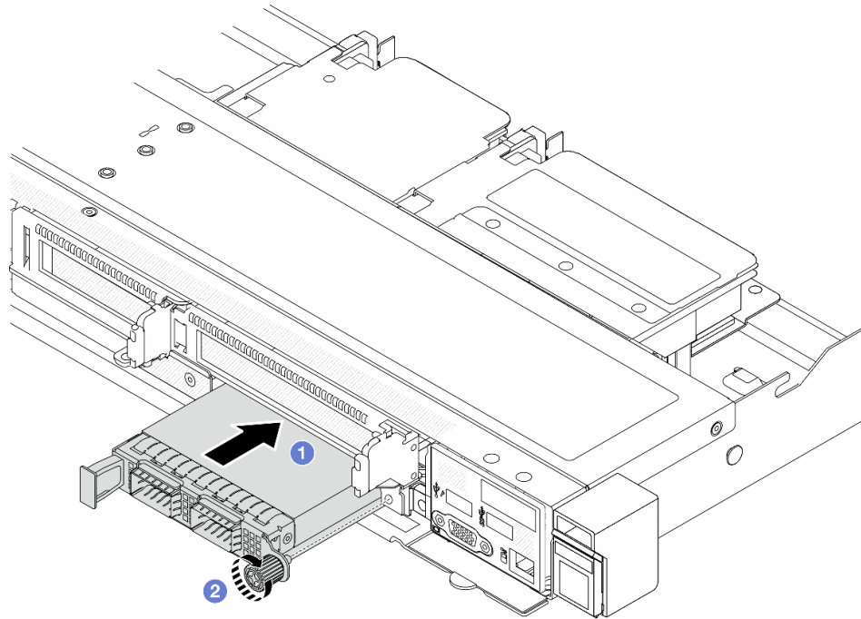
Figure 34. Installation du module OCP avant
