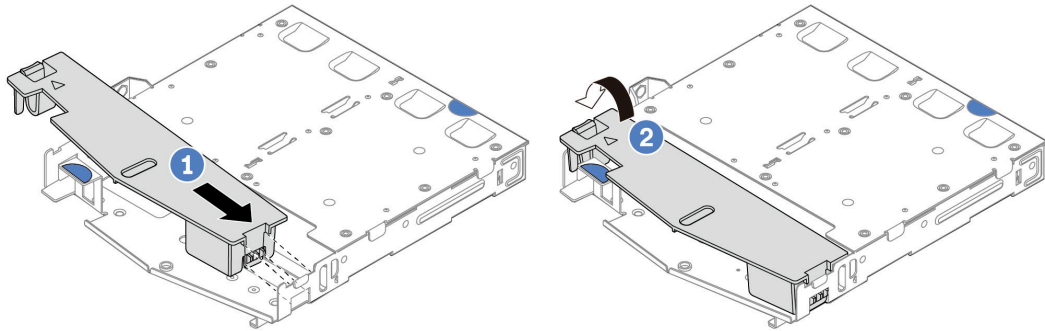
Figure 161. Installation de la grille d'aération
