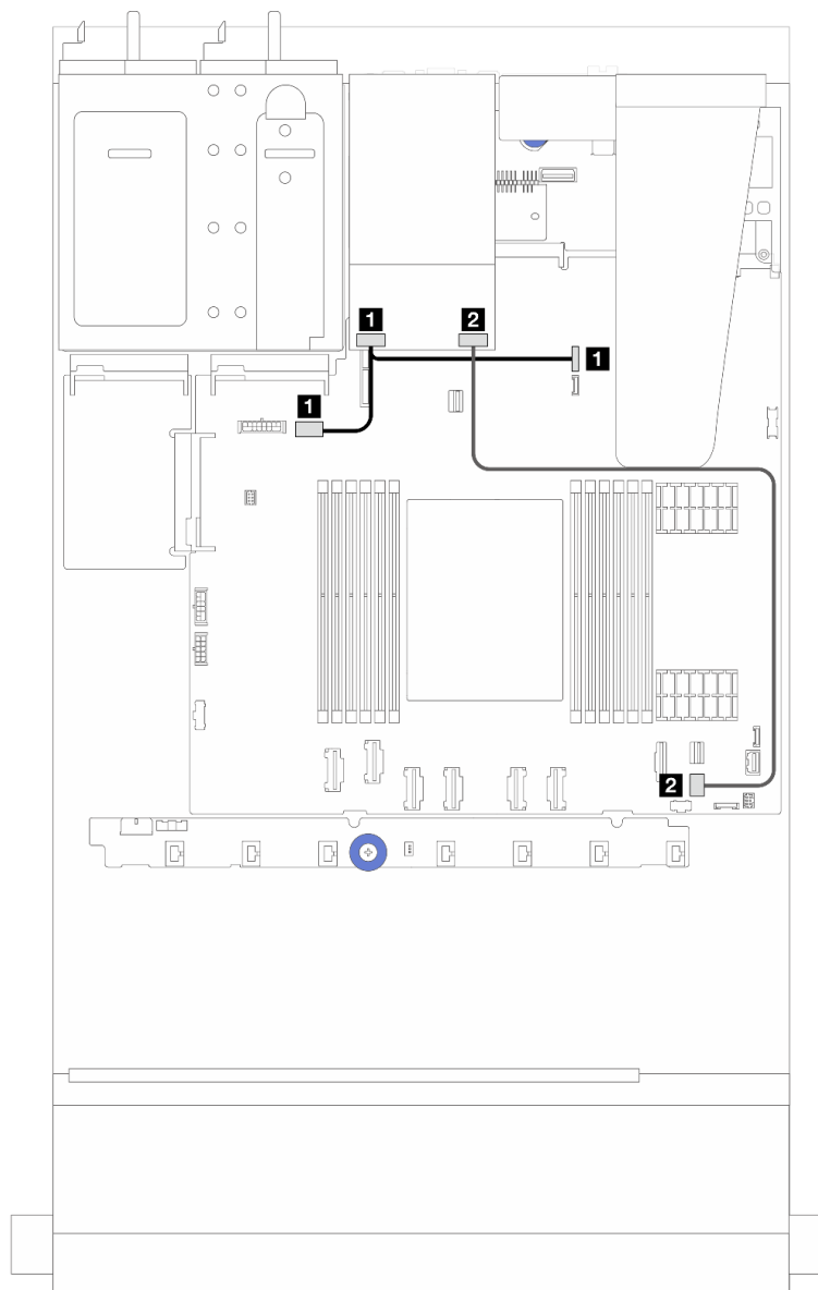
Figure 214. Cheminement des câbles SATA
