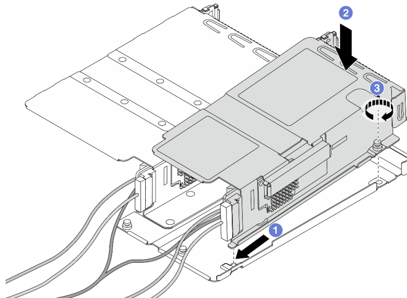
Figure 32. Assemblage des deux boîtiers de cartes mezzanines
