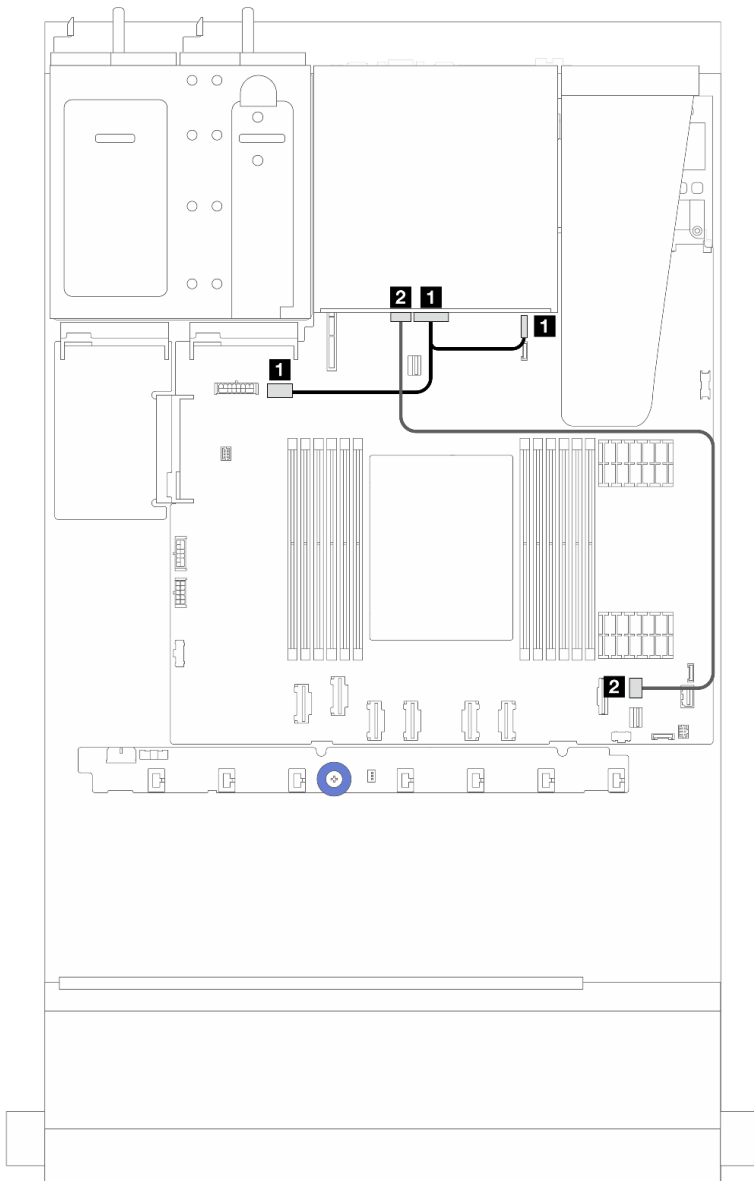
Figure 213. Cheminement des câbles du fond de panier d'unité SATA arrière 2 x 2,5 pouces
