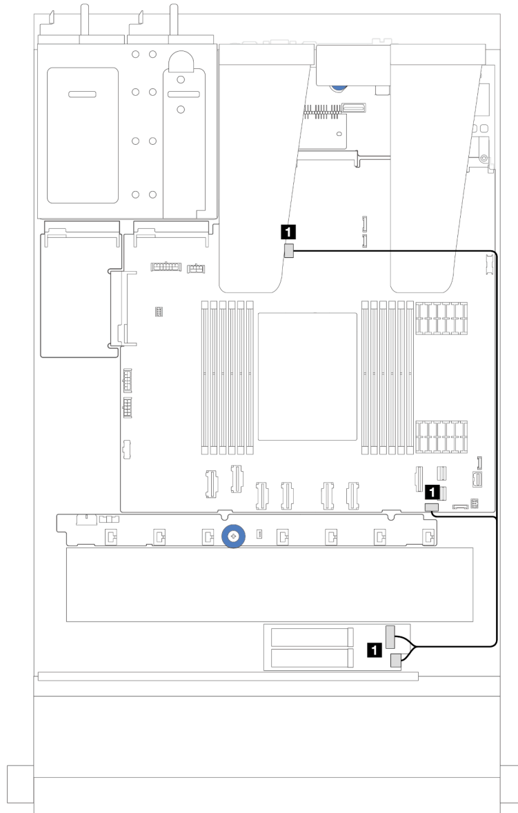
Figure 222. Cheminement des câbles pour le ThinkSystem M.2 NVMe 2-Bay RAID Enablement Kit
