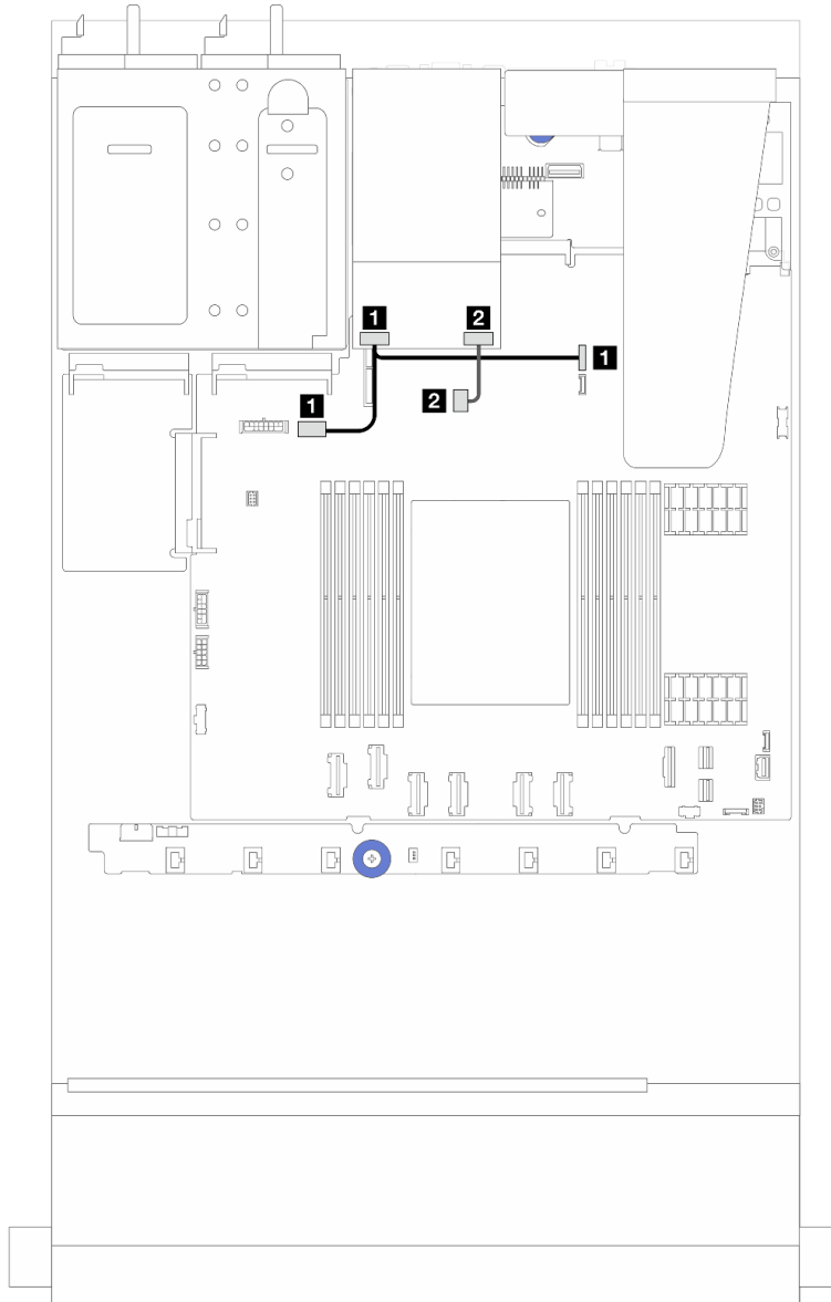
Figure 215. Cheminement des câbles NVMe
