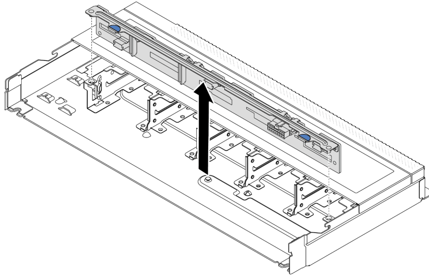
Figure 1. Retrait du fond de panier pour dix unités remplaçables à chaud 2,5 pouces
