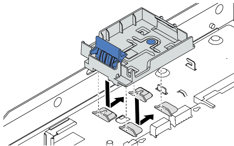
Figure 112. Installation du support de module d'alimentation flash RAID
