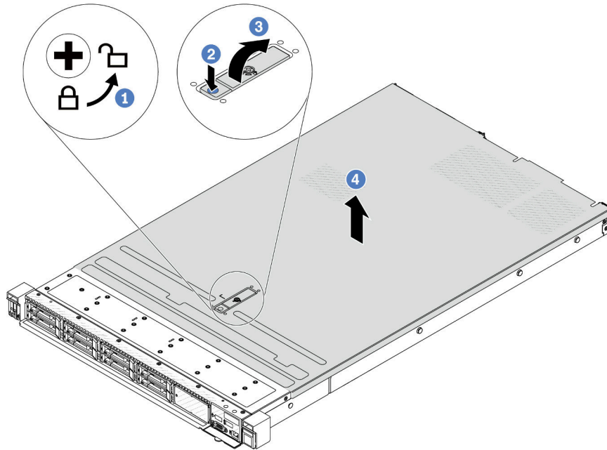
Figure 187. Retrait du carter supérieur
