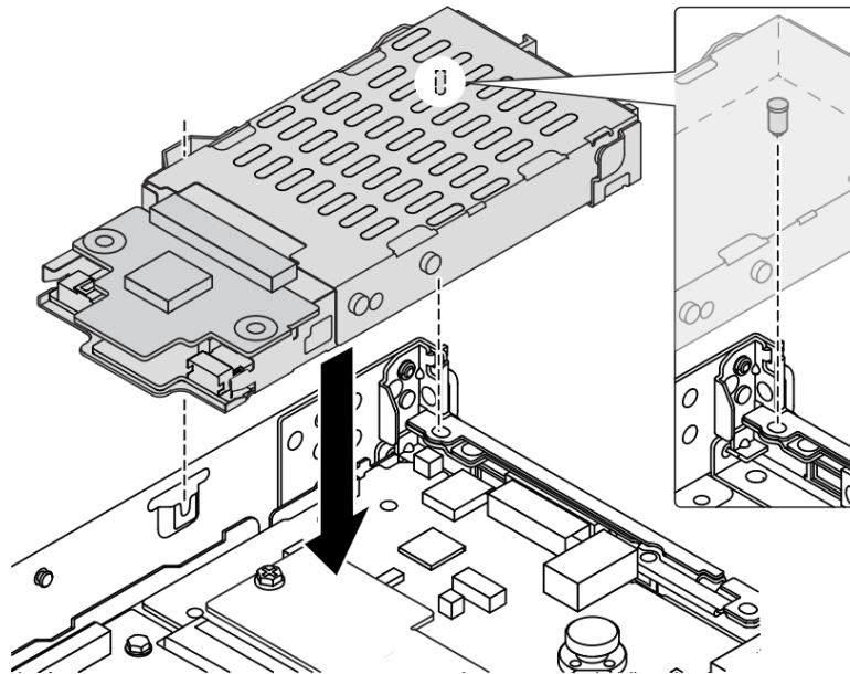
Figure 165. Installation du boîtier d'unité remplaçable à chaud arrière
