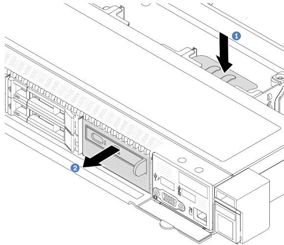
Figure 40. Retrait du bloc du panneau de diagnostics intégré
