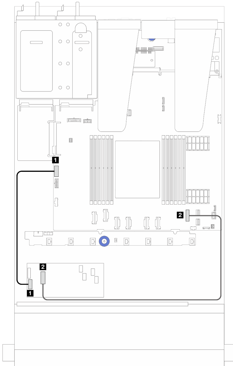
Figure 200. Câbles d'alimentation et d'entrée des adaptateurs RAID/HBA CFF Gen 3
