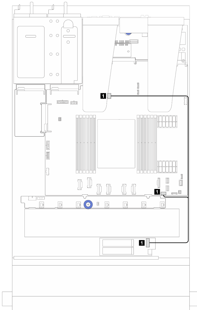
Figure 225. Cheminement des câbles pour le ThinkSystem M.2 RAID B540i-2i SATA/NVMe Enablement Kit
