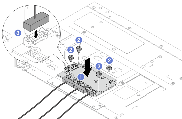
Figure 36. Installation de la carte d'interposeur OCP avant
