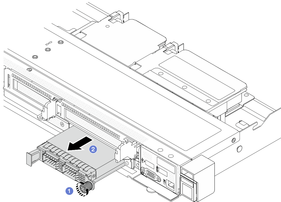
Figure 33. Retrait du module OCP avant
