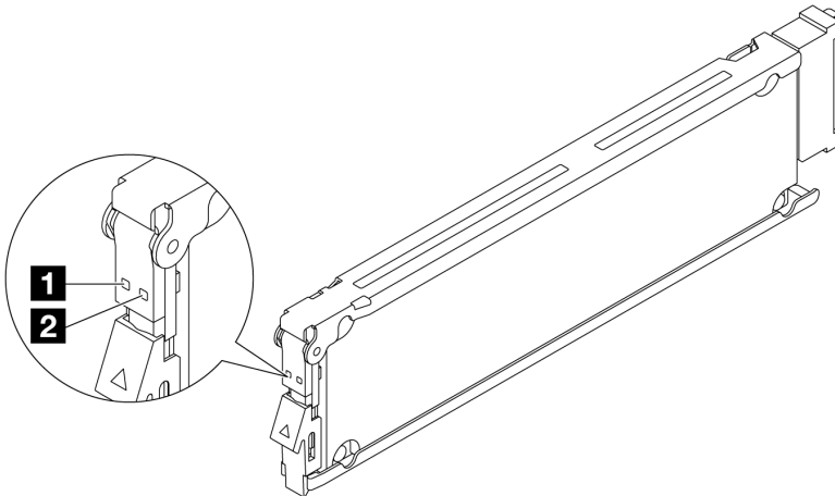
Figure 256. Voyants sur les unités EDSFF
