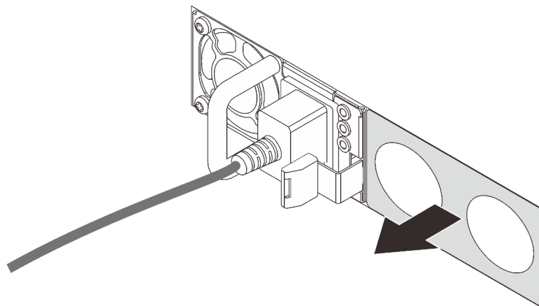
Figure 70. Retrait de l'obturateur du bloc d'alimentation remplaçable à chaud
