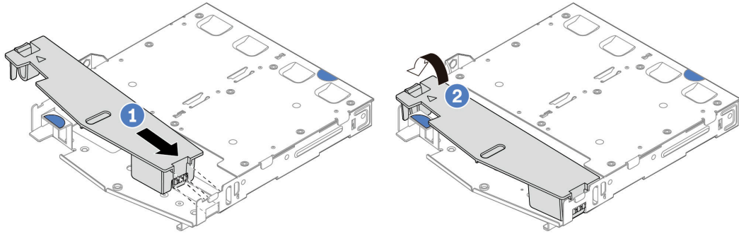
Figure 8. Installation de la grille d'aération
