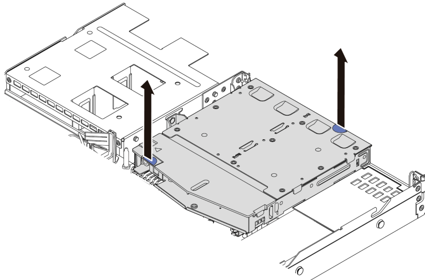
Figure 158. Retrait du boîtier d'unité remplaçable à chaud arrière
