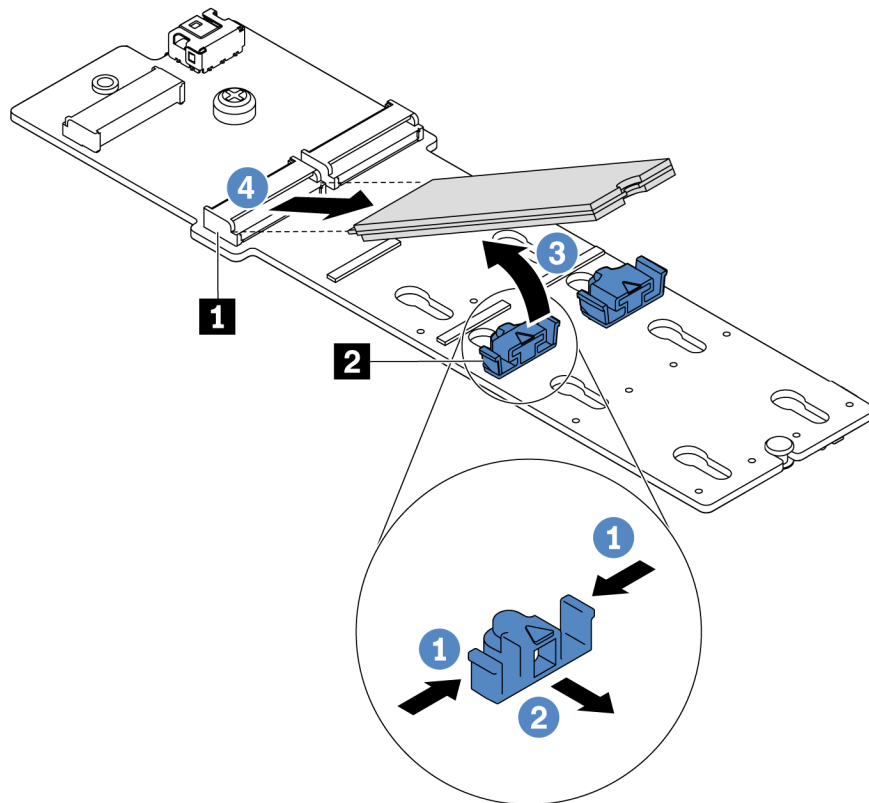
Figure 79. Retrait d'une unité M.2
