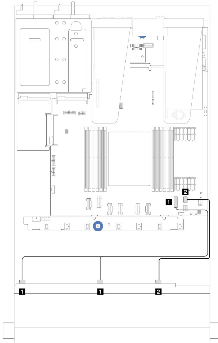
Figure 242. Cheminement des câbles pour la configuration SATA intégrée de 6 unités SAS/SATA avant et de 4 baies d'unité AnyBay avant
