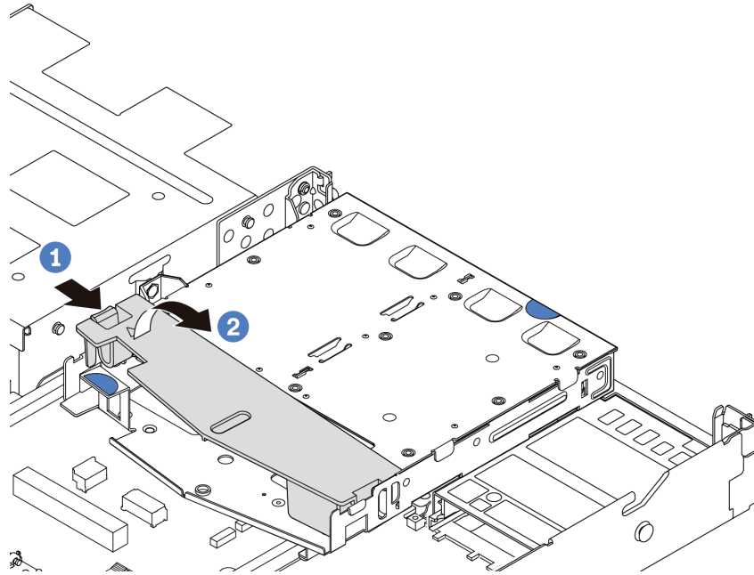
Figure 5. Retrait de la grille d'aération
