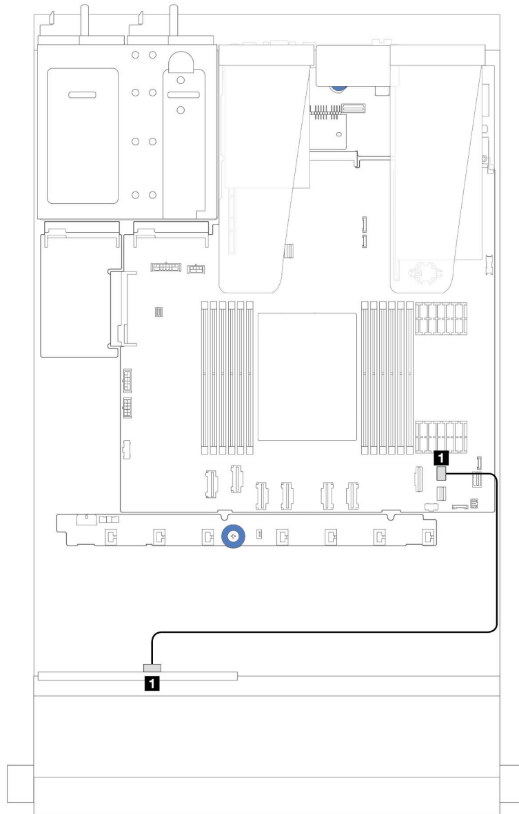
Figure 229. Cheminement des câbles pour la configuration intégrée avec des baies d'unité SAS/SATA avant 4 x 2,5 pouces
