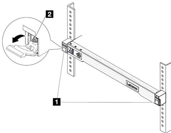
Figure 51. Dégagement du serveur de l'armoire
