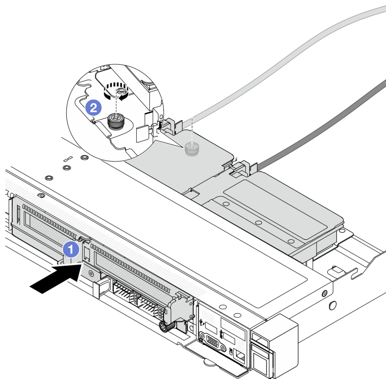
Figure 24. Installation du boîtier de la carte mezzanine avant
