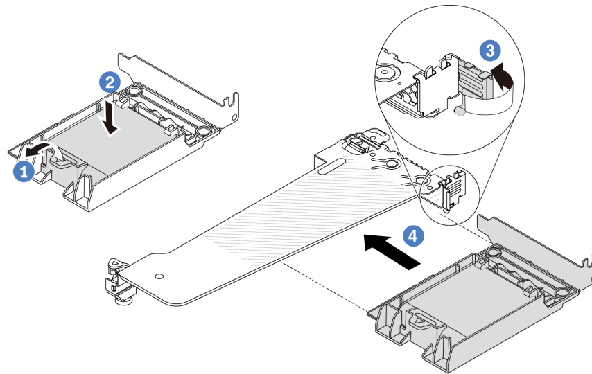
Figure 115. Installation du module d'alimentation flash RAID sur l'assemblage de cartes mezzanines
