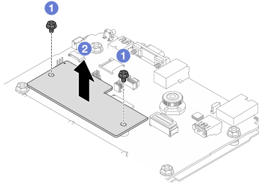
Figure 178. Retrait du Module de microprogramme et de sécurité RoT
