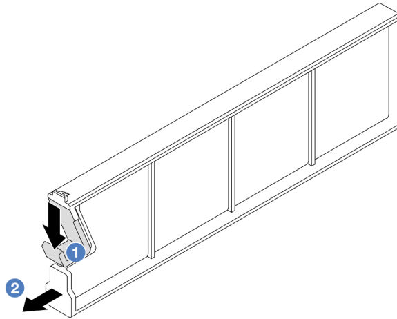
Figure 64. Retrait d'un obturateur d'unité EDSFF
