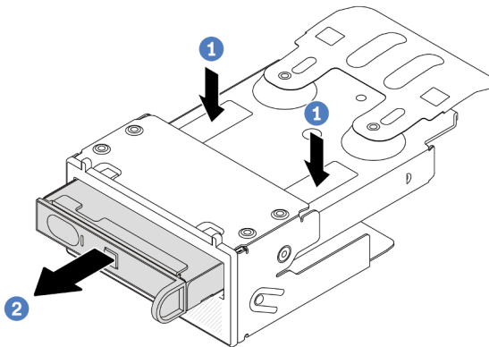
Figure 41. Retrait du panneau de diagnostics intégré
