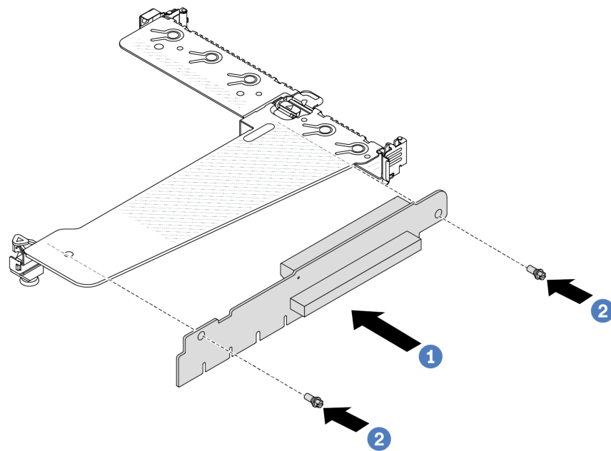
Figure 151. Installation d'une carte mezzanine
