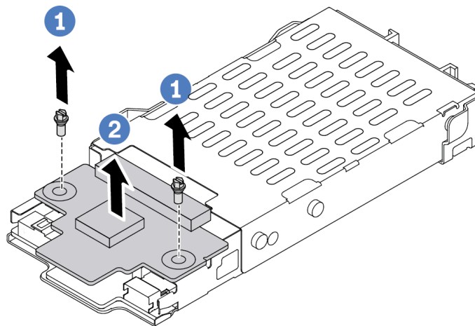
Figure 9. Retrait du fond de panier d'unité 7 mm (haut)
