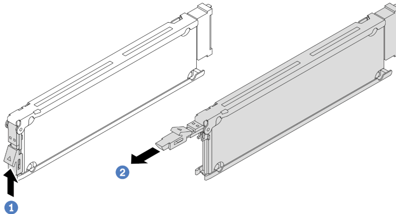
Figure 63. Retrait de l'unité EDSFF
