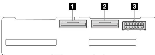
Figure 195. Fond de panier NVMe 4 x 2,5 pouces
