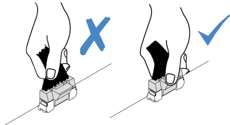
Figure 74. Déconnexion des câbles du bloc carte mère
