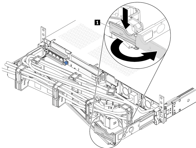
Figure 67. Ajustement du bras de routage des câbles
