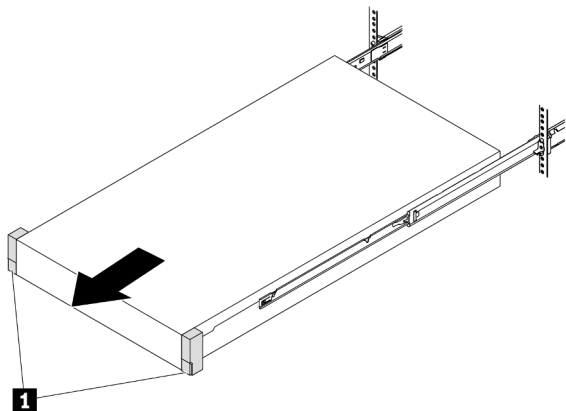
Figure 52. Extraction du serveur
