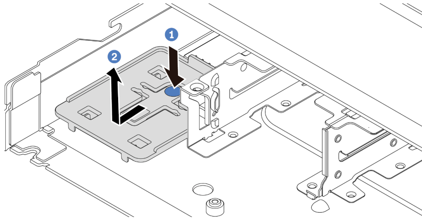
Figure 106. Retrait du plateau
