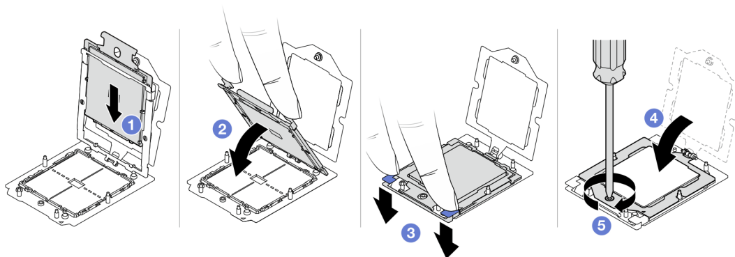
Figure 96. Installation d'un processeur
