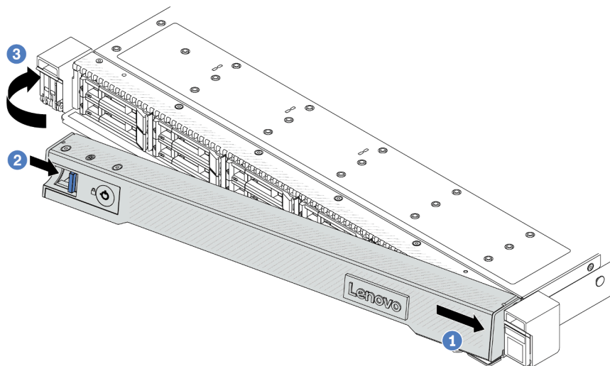
Figure 169. Installation du panneau de sécurité
