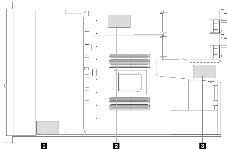
Figure 103. Modules d'alimentation flash RAID sur le châssis
