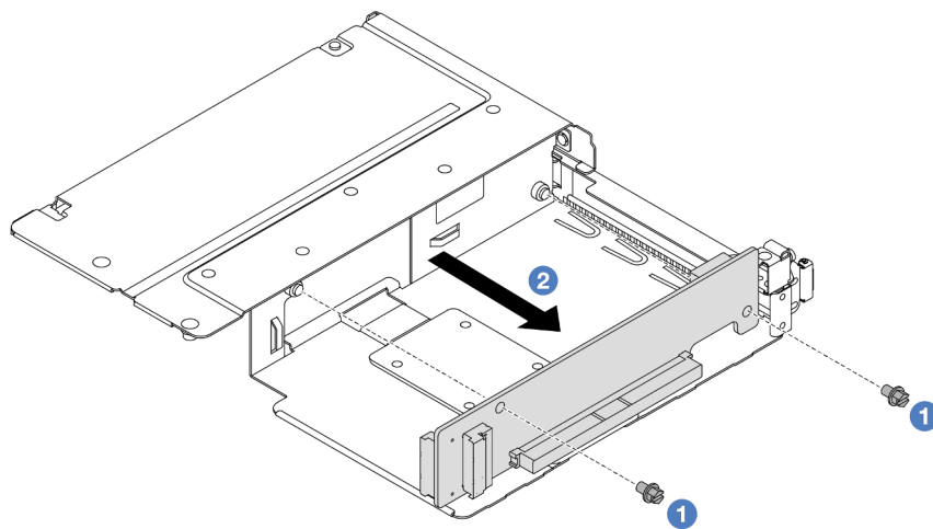
Figure 28. Retrait de la carte mezzanine du boîtier pleine hauteur
