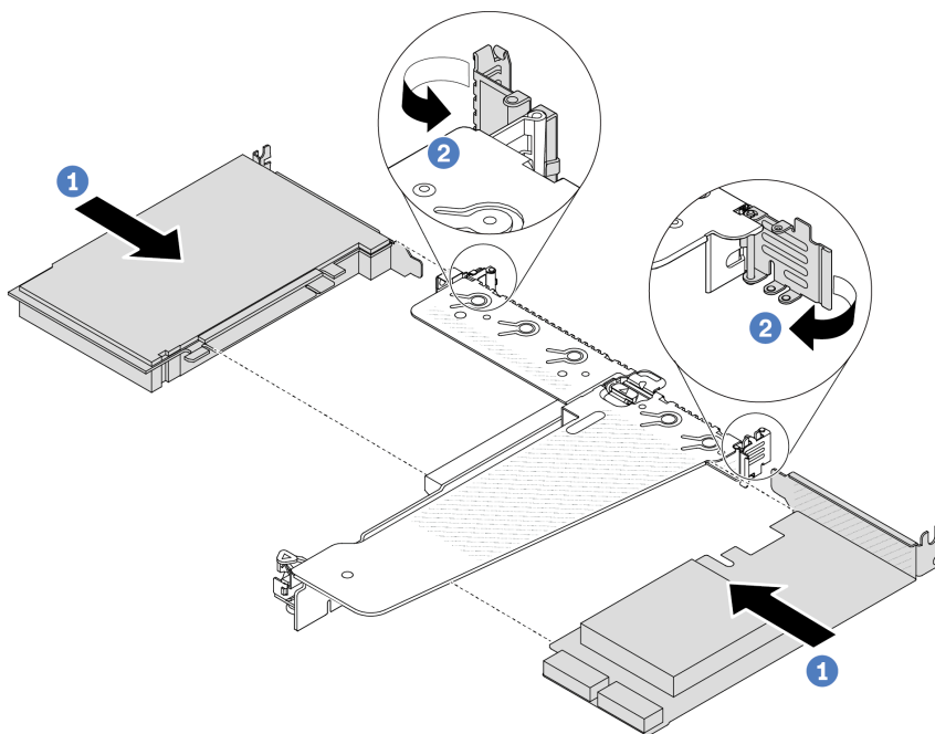
Figure 88. Installation de l'adaptateur PCIe dans l'assemblage de cartes mezzanines LP-FH
