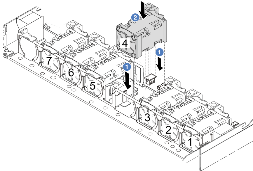
Figure 186. Installation du ventilateur système
