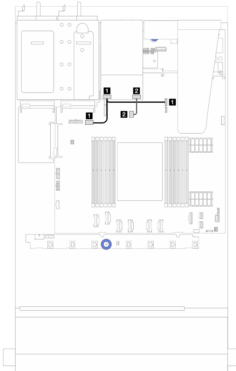
Figure 218. Cheminement des câbles pour les fonds de panier d'unité 7 mm SATA/NVMe RAID à 2 baies
