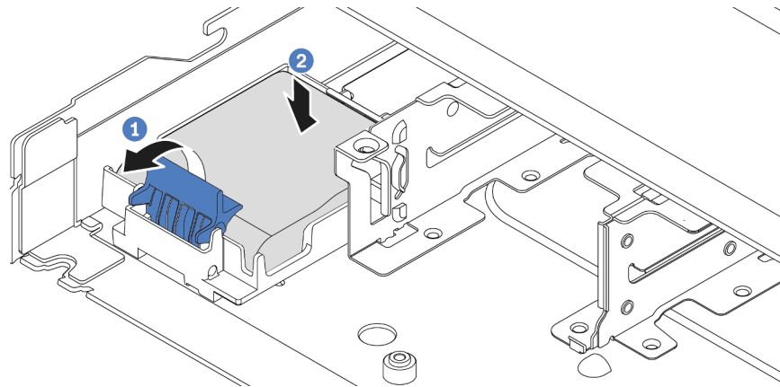
Figure 108. Installation du module d'alimentation flash RAID sur le châssis
