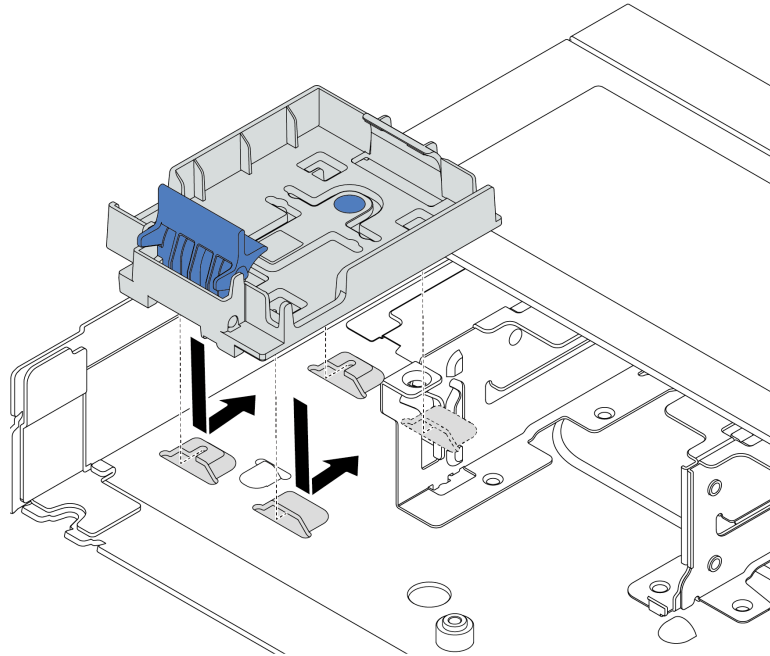
Figure 107. Installation du support de module d'alimentation flash RAID
