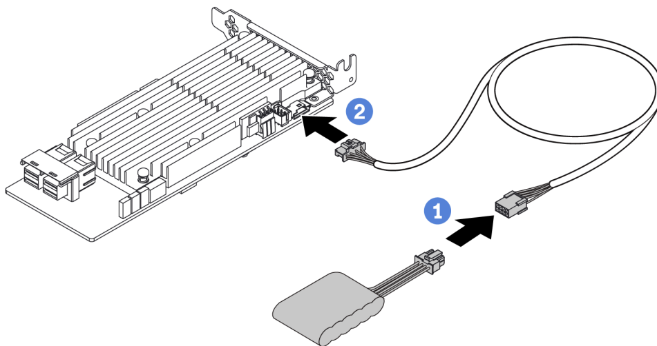
Figure 211. Cheminement des câbles d'alimentation du module d'alimentation flash RAID
