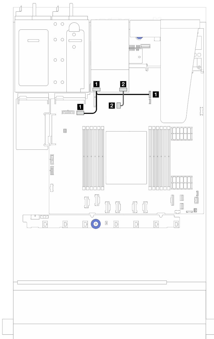
Figure 217. Cheminement des câbles pour les fonds de panier d'unité 7 mm NVMe RAID à 2 baies
