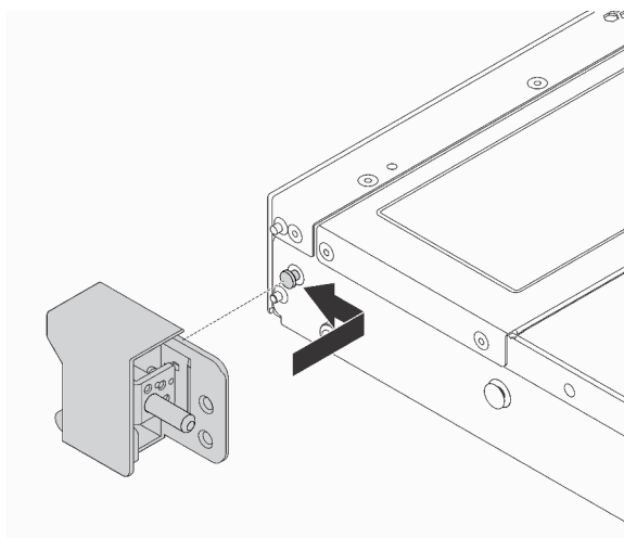
Figure 101. Installation du taquet d'armoire
