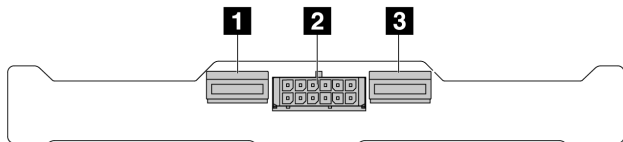
Figure 198. Fond de panier NVMe 2 x 2,5" arrière
