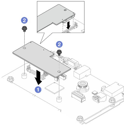
Figure 179. Installation du Module de microprogramme et de sécurité RoT
