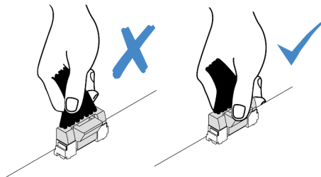
Figure 163. Déconnexion des câbles du bloc carte mère
