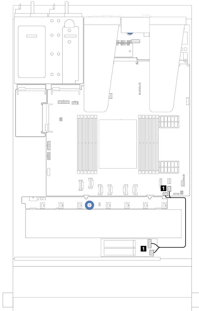
Figure 220. Cheminement des câbles SATA
