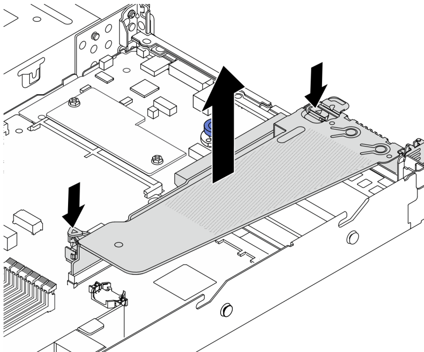
Figure 171. Retrait du support de carte mezzanine
