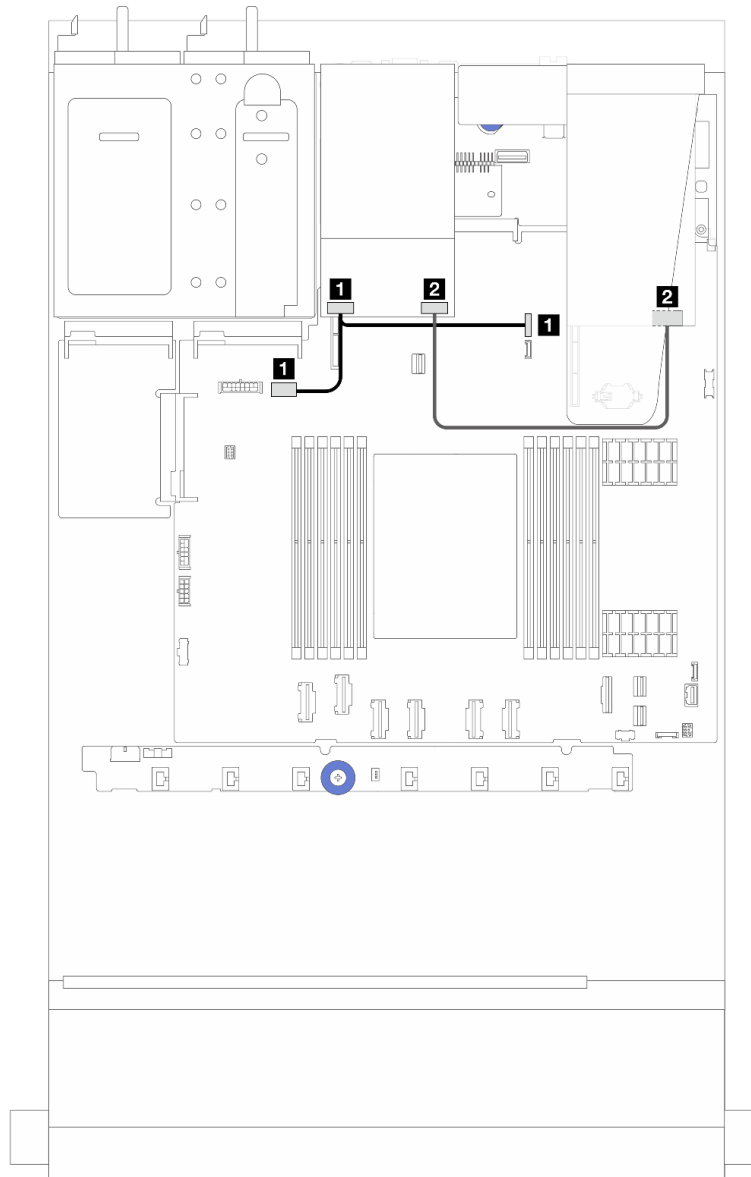
Figure 216. Cheminement des câbles RAID (avec un adaptateur RAID SFF Gen 3/Gen 4 8i)
