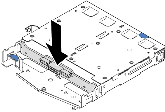
Figure 160. Installation du fond de panier arrière
