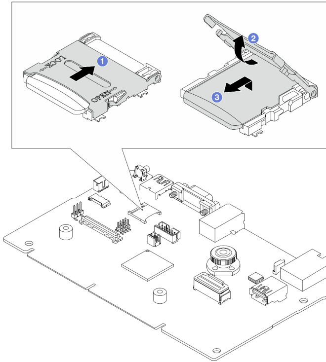
Figure 85. Retrait d'une carte MicroSD
