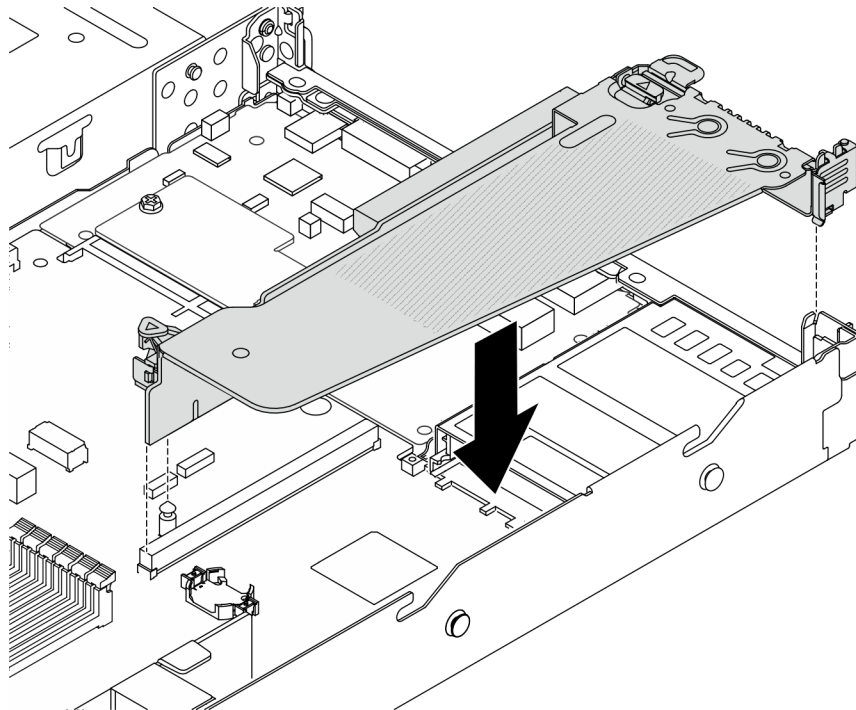
Figure 176. Installation de l'assemblage de cartes mezzanines
