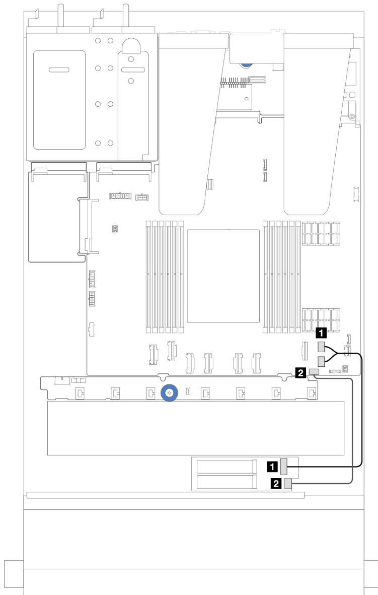
Figure 223. Cheminement des câbles SATA/NVMe
