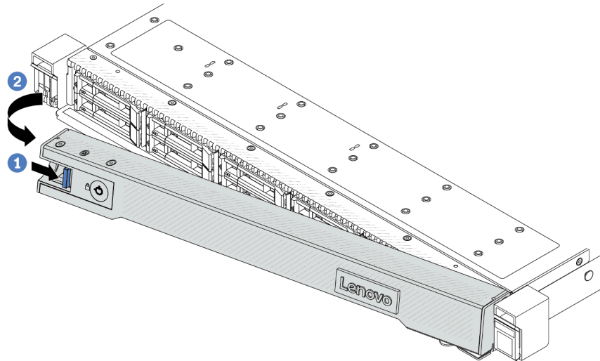
Figure 167. Retrait du panneau de sécurité
