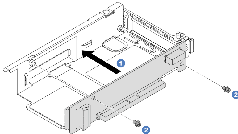
Figure 29. Installation de la carte mezzanine dans un boîtier extra-plat
