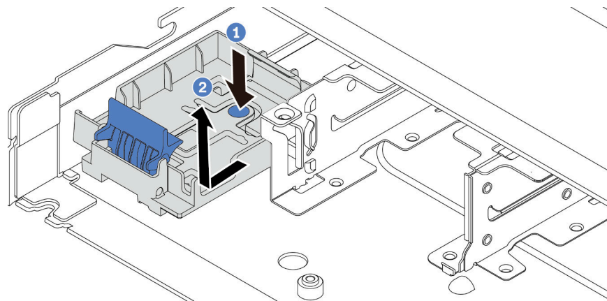
Figure 105. Retrait du support du module d'alimentation flash RAID
