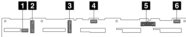
Figure 190. 6 fonds de panier SAS/SATA + 4 fonds de panier AnyBay
