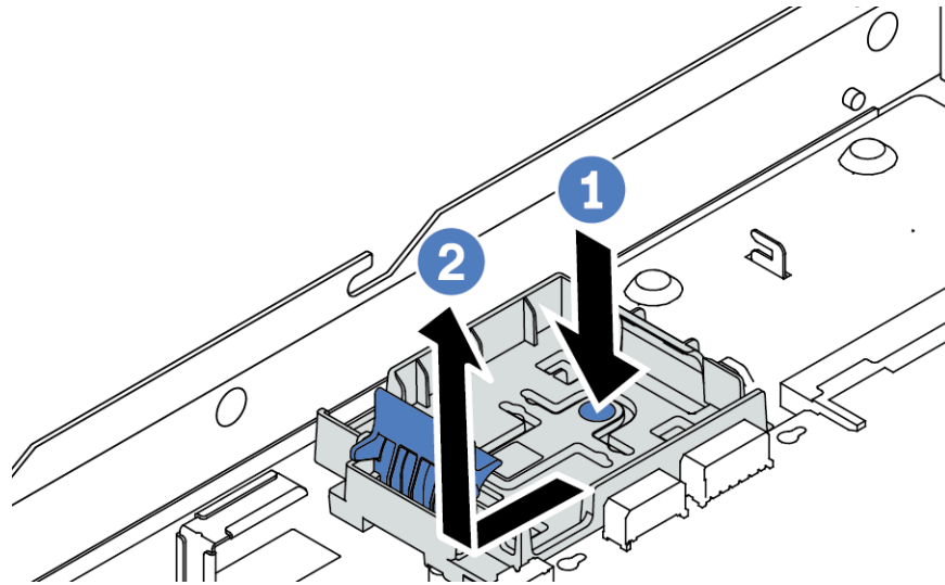
Figure 110. Retrait du support du module d'alimentation flash RAID
