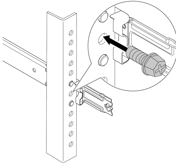
Figure 58. Fixation du serveur à l'arrière de l'armoire
