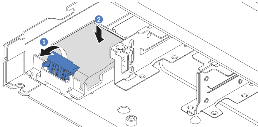
Figure 113. Installation du module d'alimentation flash RAID sur le plateau de la carte mère
