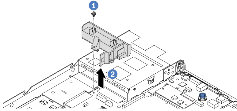
Figure 89. Retrait d'une grille d'aération du bloc d'alimentation
