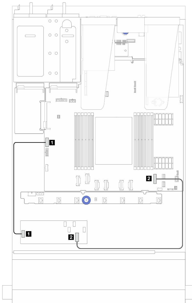
Figure 201. Câbles d'alimentation et d'entrée des adaptateurs RAID CFF Gen 4
