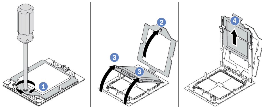
Figure 93. Retrait d'un processeur
