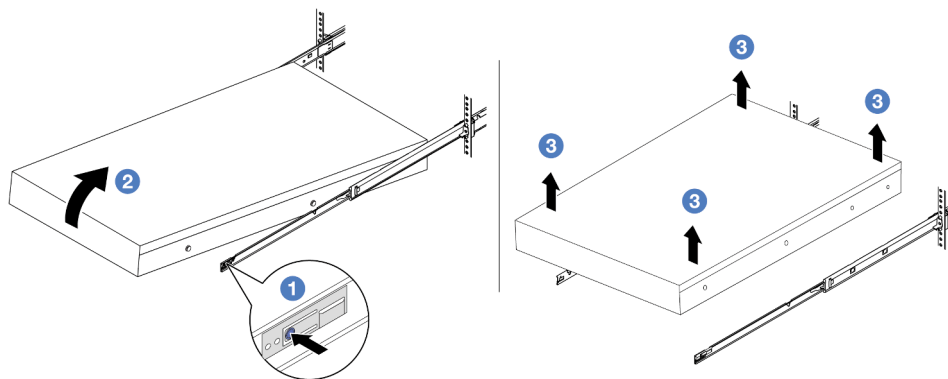
Figure 54. Retrait du serveur de l'armoire.
