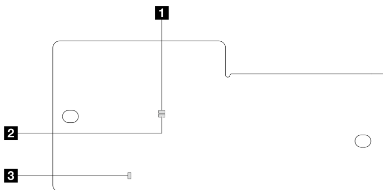
Figure 261. Voyants du module de microprogramme et de sécurité RoT
