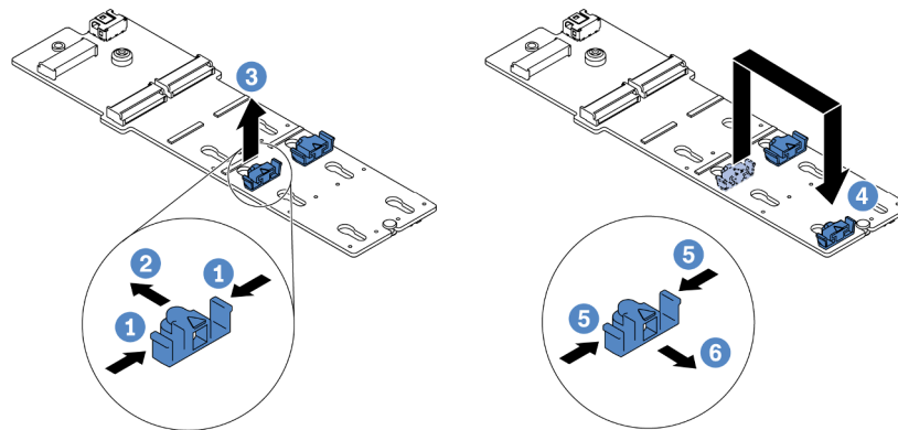
Figure 81. Ajustement du dispositif de retenue M.2
