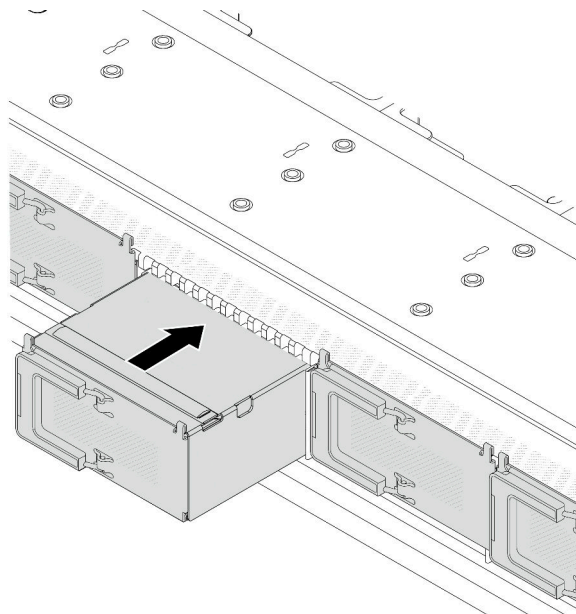
Figure 16. Installation du boîtier d'unités EDSFF
