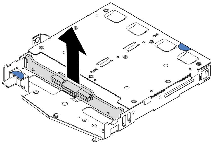
Figure 6. Retrait du fond de panier d'unité 2,5 pouces arrière
