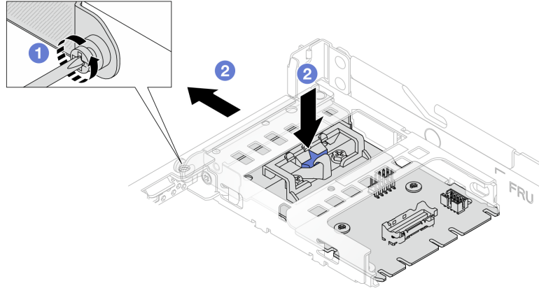
Figure 37. Retrait de la carte d'interposeur OCP arrière
