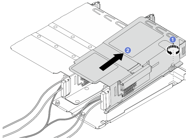
Figure 25. Séparation des deux boîtiers
