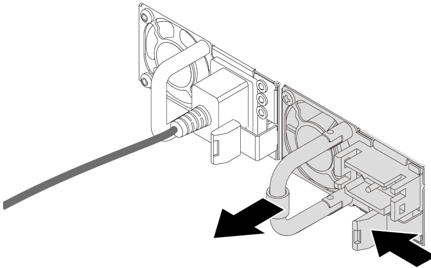
Figure 68. Retrait du bloc d'alimentation
