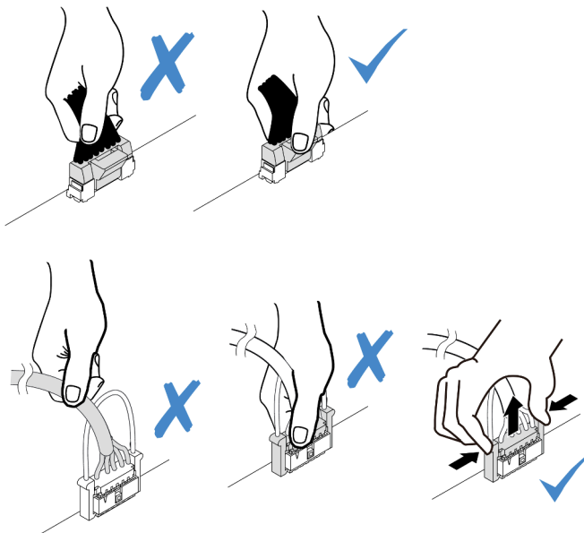
Figure 39. Déconnexion des câbles du bloc carte mère
