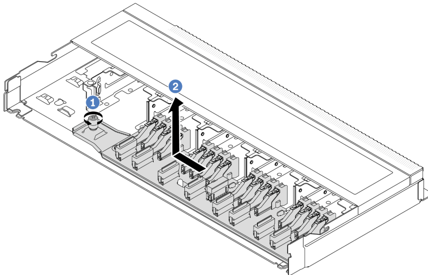
Figure 3. Retrait du fond de panier pour 16 unités EDSFF
