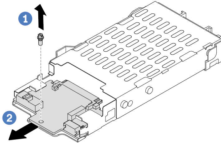
Figure 10. Retrait du fond de panier d'unité 7 mm (bas)
