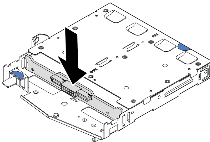
Figure 7. Installation du fond de panier arrière
