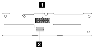
Figure 194. Fond de panier SAS/SATA 4 x 2,5 pouces
