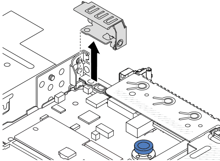
Figure 150. Retrait du support mural arrière
