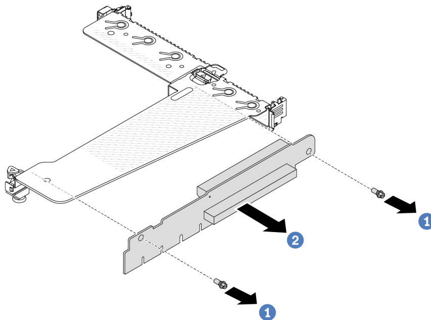
Figure 149. Retrait de la carte mezzanine
