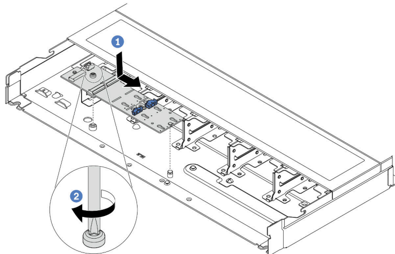
Figure 83. Installation du fond de panier M.2
