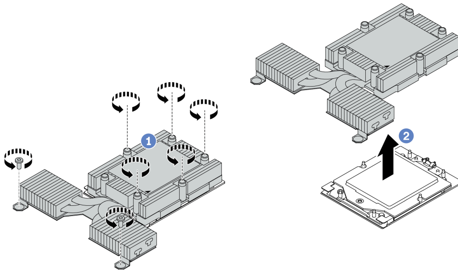
Figure 92. Retrait d'un dissipateur thermique à refroidissement par air
