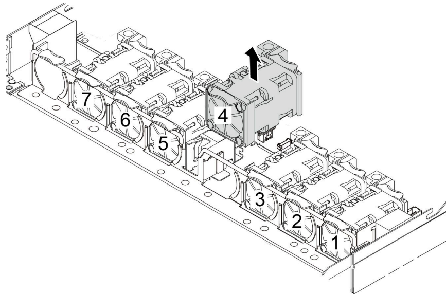
Figure 185. Retrait du ventilateur système
