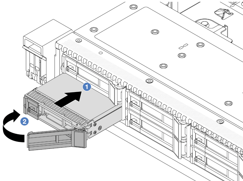
Figure 61. Installation d'une unité remplaçable à chaud
