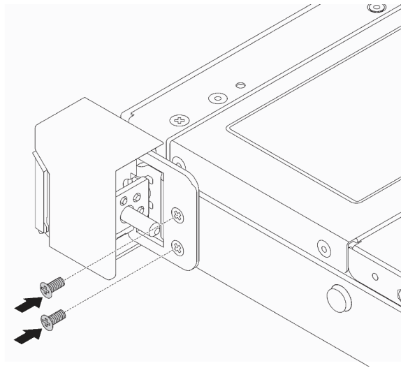
Figure 102. Installation des vis du taquet d'armoire
