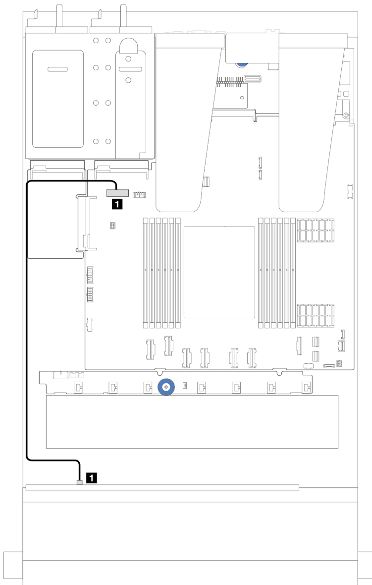
Figure 226. Connexion du câble d'alimentation du fond de panier pour les fonds de panier d'unité 8 ou 10 x 2,5 pouces
