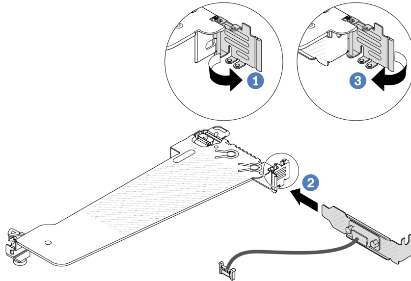
Figure 175. Installation du module de port série
