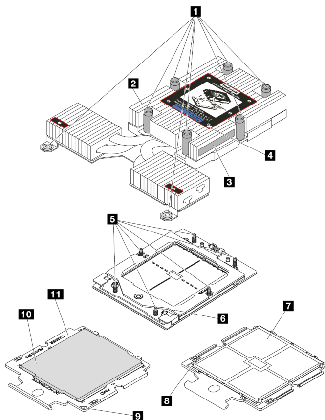
Figure 91. Composants du processeur et du dissipateur thermique
