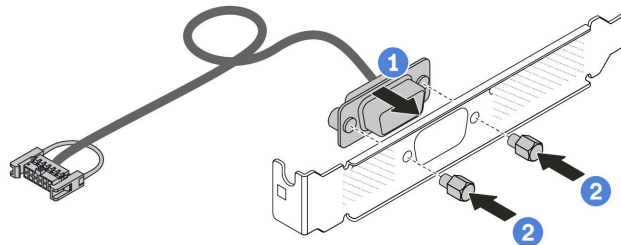
Figure 174. Assemblage du module de port série
