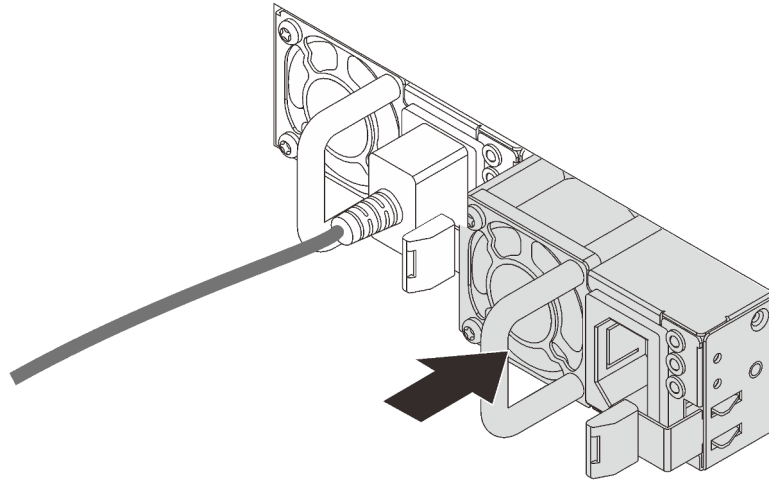
Figure 71. Installation du bloc d'alimentation remplaçable à chaud
