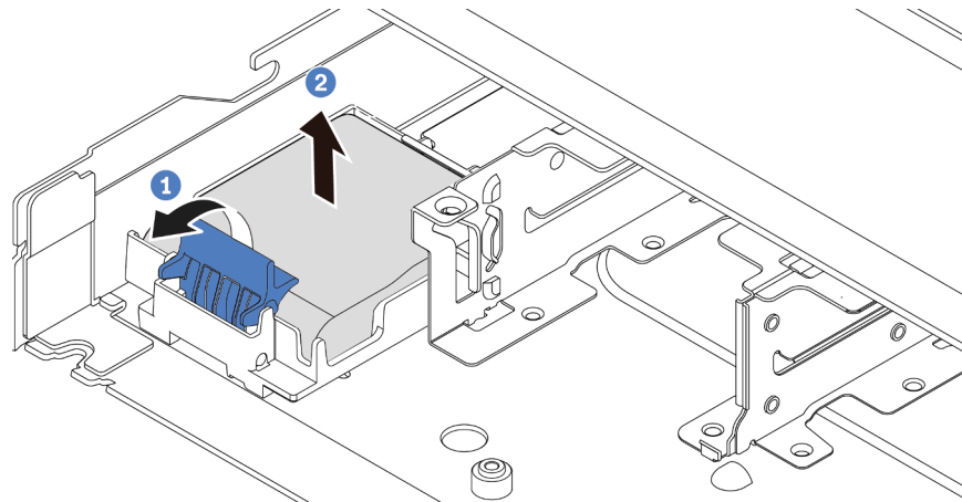
Figure 104. Retrait du module d'alimentation flash RAID du châssis
