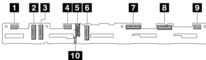
Figure 192. Fond de panier AnyBay 10 X 2,5 pouces (Gen 5)
