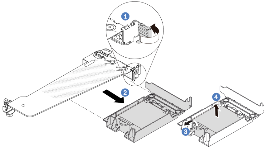
Figure 114. Retrait du bloc du module d'alimentation flash RAID de la carte mezzanine
