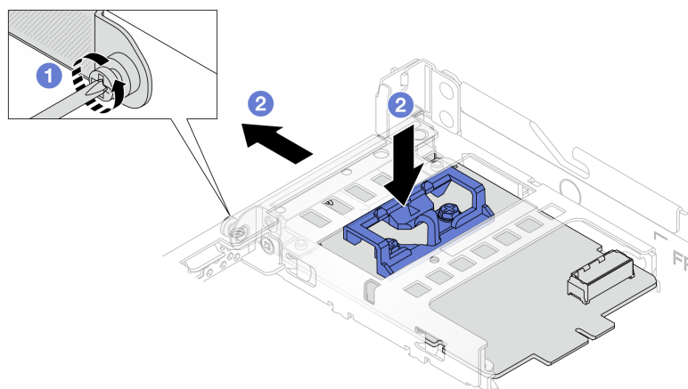
Figure 75. Retrait de l'adaptateur NIC de gestion
