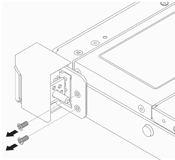
Figure 99. Retrait des vis du taquet d'armoire
