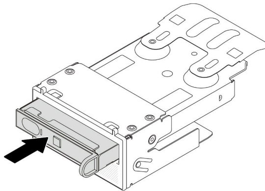
Figure 43. Installation du panneau de diagnostics intégré dans son assemblage
