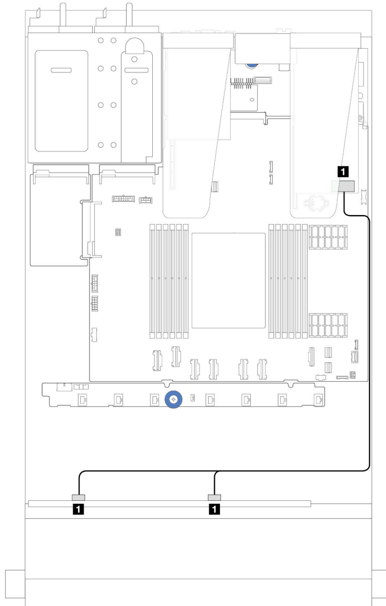
Figure 236. Cheminement des câbles pour 8 baies d'unité SAS/SATA avant 2,5" et un adaptateur RAID SFF 8i ou 16i (Gen 4)
