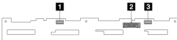
Figure 193. Fond de panier SAS/SATA 8 x 2,5
