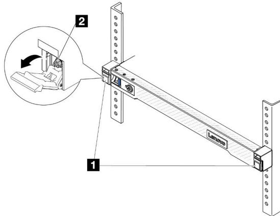
Figure 59. Fixation du serveur à l'avant de l'armoire
