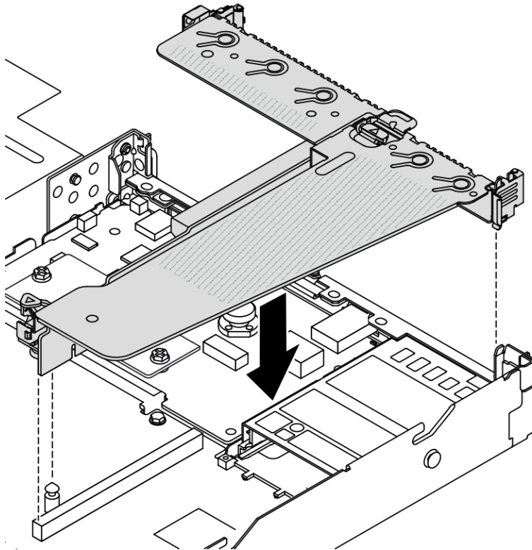
Figure 152. Installation de l'assemblage de cartes mezzanines
