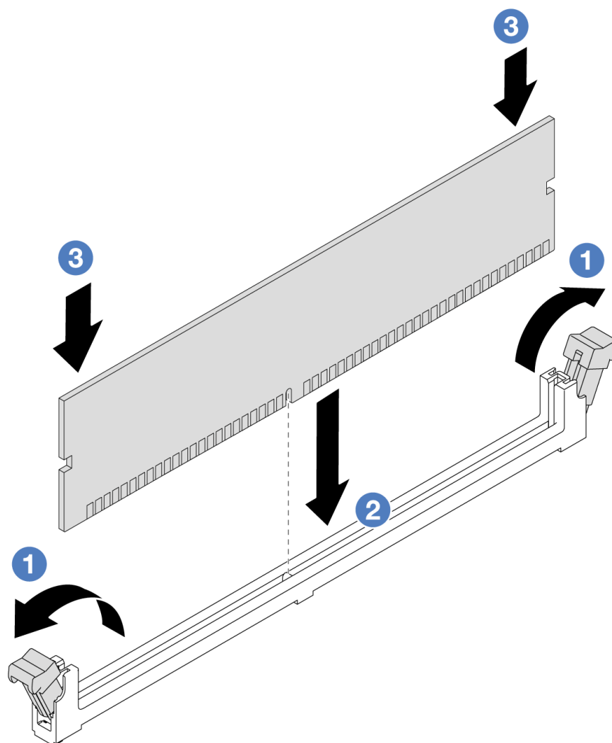
Figure 78. Installation du module de mémoire
