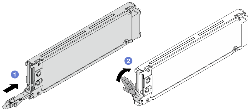
Figure 65. Installation d'une unité EDSFF
