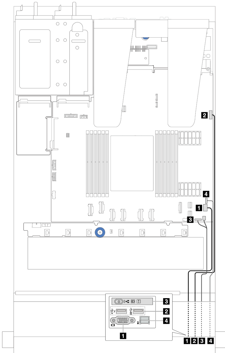
Figure 202. Cheminement des câbles pour un module d'E-S avant sur le châssis 2,5 pouces
