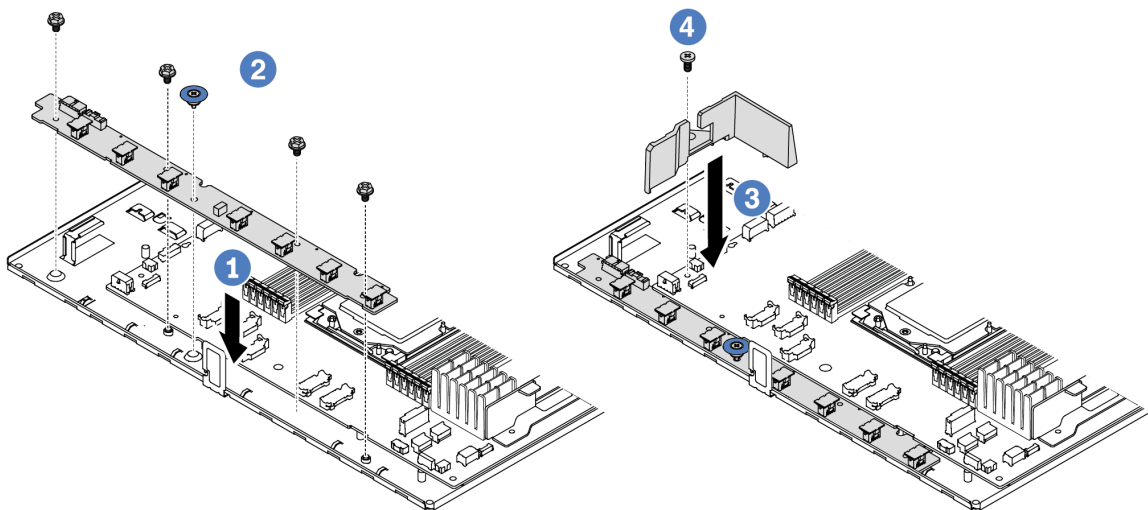
Figure 46. Installation de la carte de ventilateur
