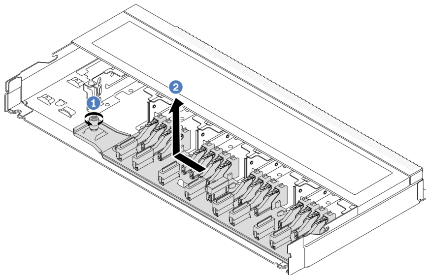
Figure 4. Installation d'un fond de panier pour 16 unités EDSFF
