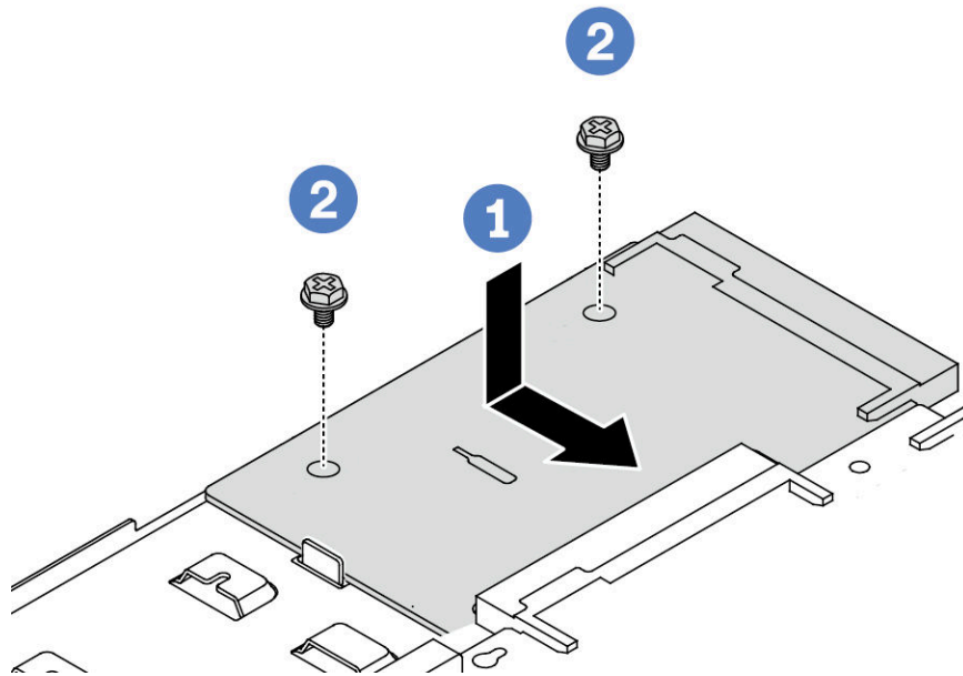
Figure 98. Installation de la carte PIB
