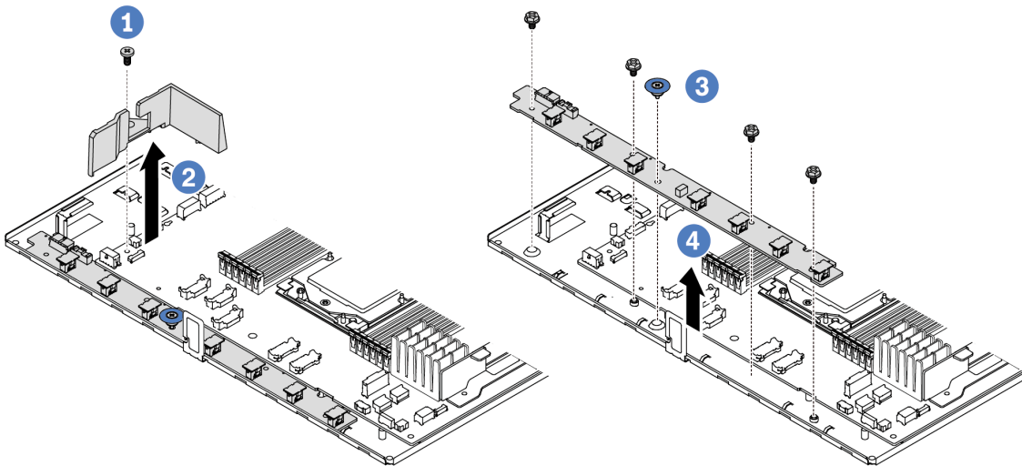
Figure 45. Retrait de la carte du ventilateur
