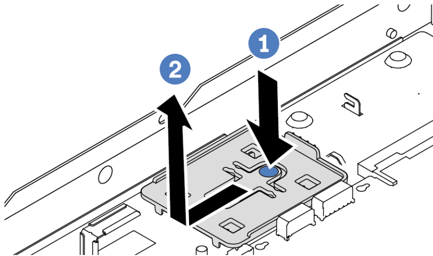
Figure 111. Retrait du plateau
