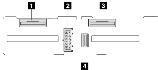
Figure 196. Fond de panier AnyBay 4 x 2,5 pouces
