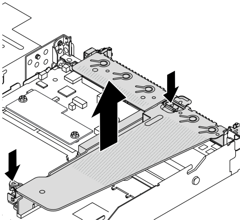
Figure 148. Retrait de l'assemblage de carte mezzanine
