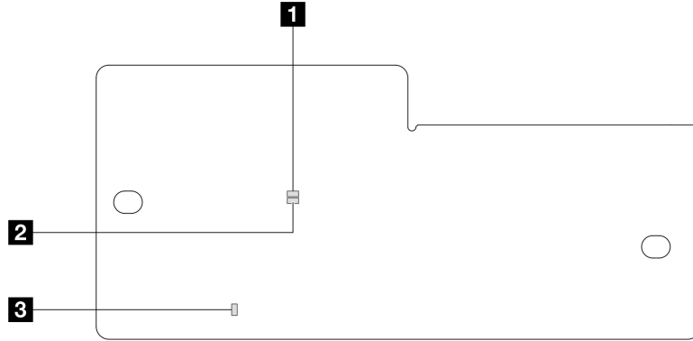
그림 22. 펌웨어 및 RoT 보안 모듈의 LED
