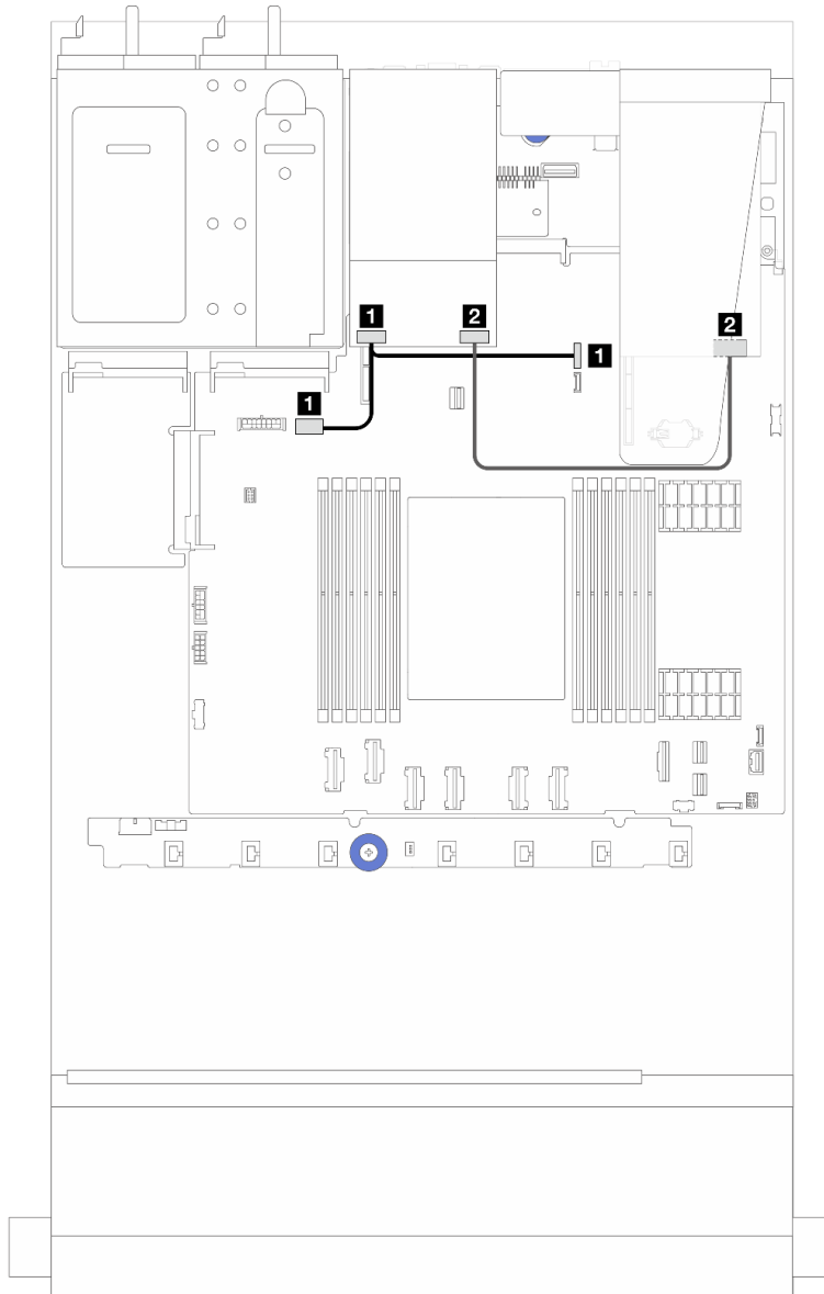
รูปภาพ 216. การเดินสาย RAID (ด้วย อะแดปเตอร์ 8i SFF RAID Gen 3/ Gen 4)
