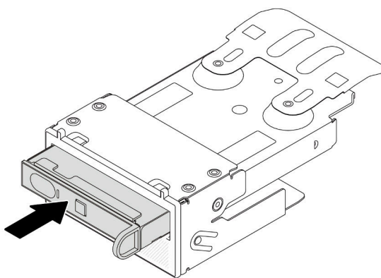
รูปภาพ 43. การติดตั้งแผงการวินิจฉัยในตัวลงในส่วนประกอบ
