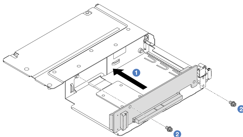
รูปภาพ 30. การติดตั้งการ์ดตัวยกกับตัวครอบแบบสูงเต็มที
