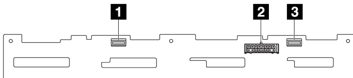
รูปภาพ 193. แบ็คเพลน SAS/SATA ขนาด 2.5 นิ้ว 8 ชุด
