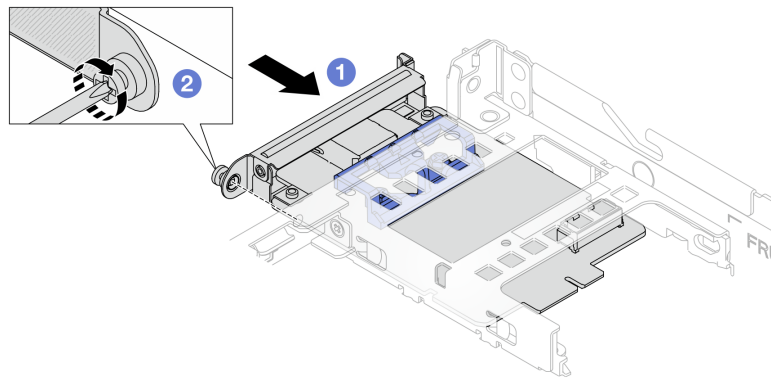
รูปภาพ 76. การติดตั้งอะแดปเตอร์ NIC การจัดการ
