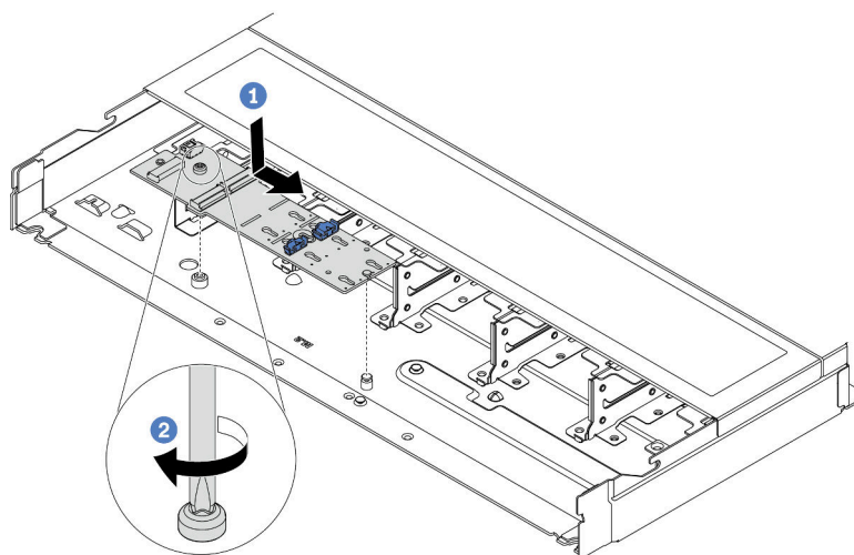
รูปภาพ 83. การติดตั้งแบ็คเพลน M.2
