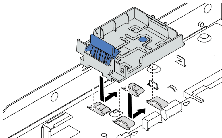
รูปภาพ 112. การติดตั้งตัวยึดโมดูลพลังงานแบบแฟลชของ RAID
