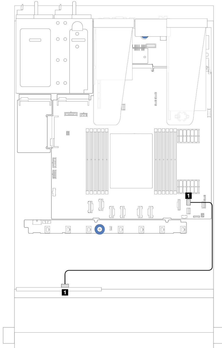
รูปภาพ 229. การเดินสายสำหรับการกำหนดค่าแบบบนแผงสำหรับช่องใส่ไดรฟ์ SAS/SATA ด้านหน้าขนาด 2.5 นิ้ว 4 ชุด
