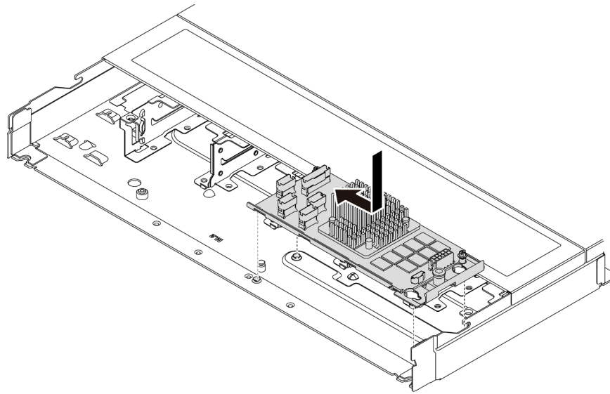
รูปภาพ 73. การติดตั้งอะแดปเตอร์ CFF HBA/RAID ภายใน
