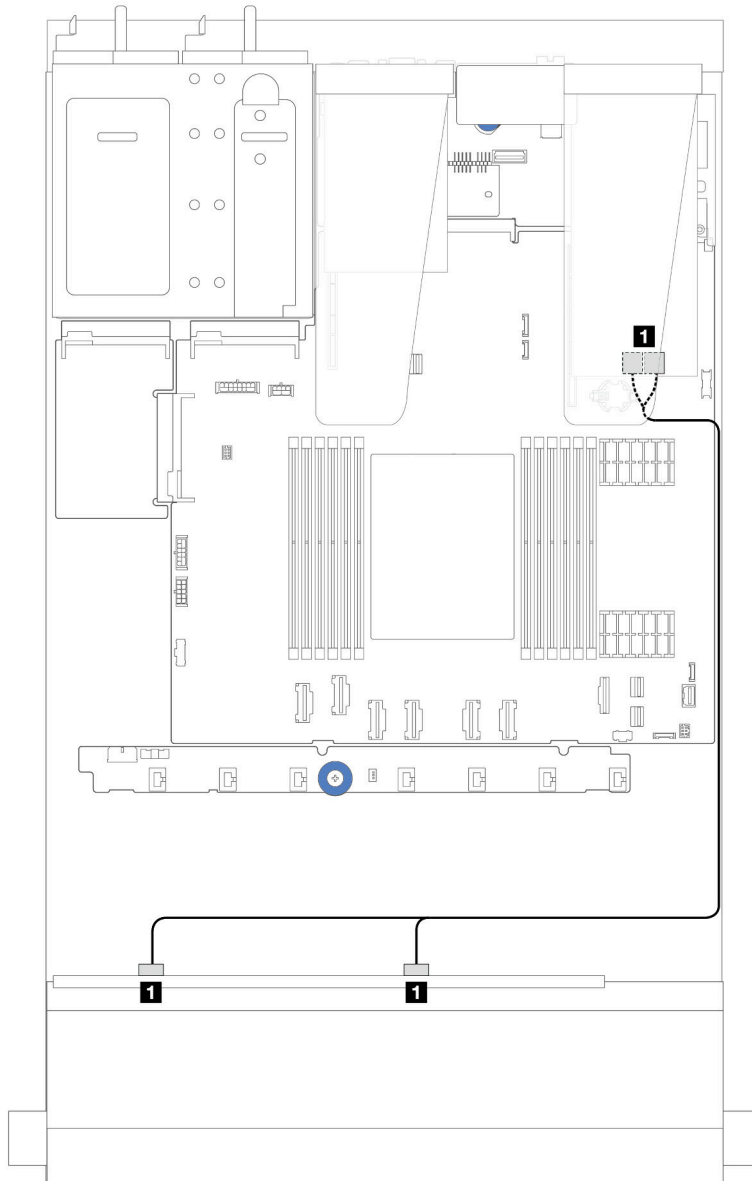
รูปภาพ 237. การเดินสายสำหรับช่องใส่ไดรฟ์ SAS/SATA ด้านหน้าขนาด 2.5 นิ้ว 8 ชุดที่มีอะแดปเตอร์ 8i หรือ 16i SFF RAID (Gen 3)
