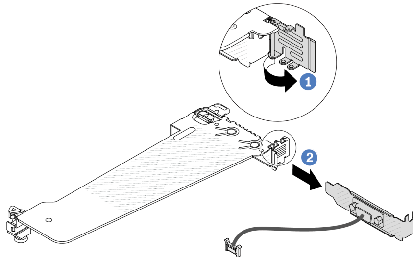
รูปภาพ 172. การถอดโครงยึดตัวยก
