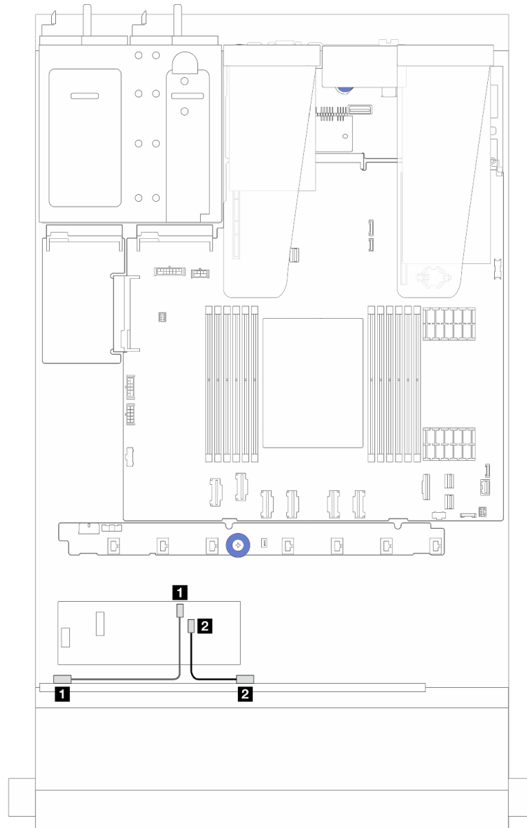
รูปภาพ 251. การเดินสายช่องใส่ไดรฟ์ SAS/SATA 6 ตัว และ AnyBay 2 ตัว และ NVMe ด้านหน้า 2 ตัว ที่มีอะแดปเตอร์ CFF RAID 8i (Gen 3)
