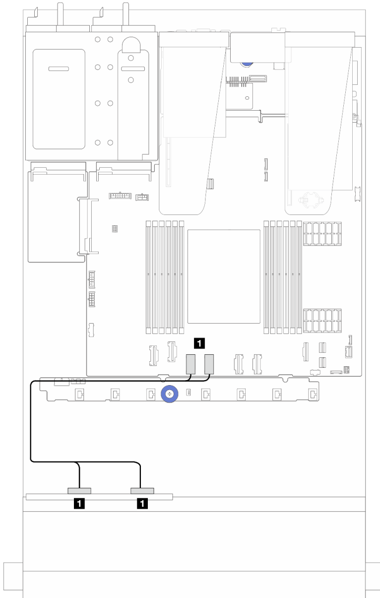
รูปภาพ 232. การเดินสายสำหรับการกำหนดค่าบนแผงของช่องใส่ไดรฟ์ NVMe ด้านหน้าขนาด 2.5 นิ้ว 4 ชุด (โดยใช้แบ็คเพลน AnyBay ขนาด 2.5 นิ้ว 4 ตัว (Gen 5))
