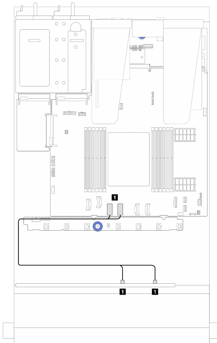
รูปภาพ 241. การเดินสายการกำหนดค่า NVMe บนแผงของไดรฟ์ SAS/SATA ด้านหน้า 6 ชุด และช่องใส่ไดรฟ์ AnyBay ด้านหน้า 4 ช่อง
