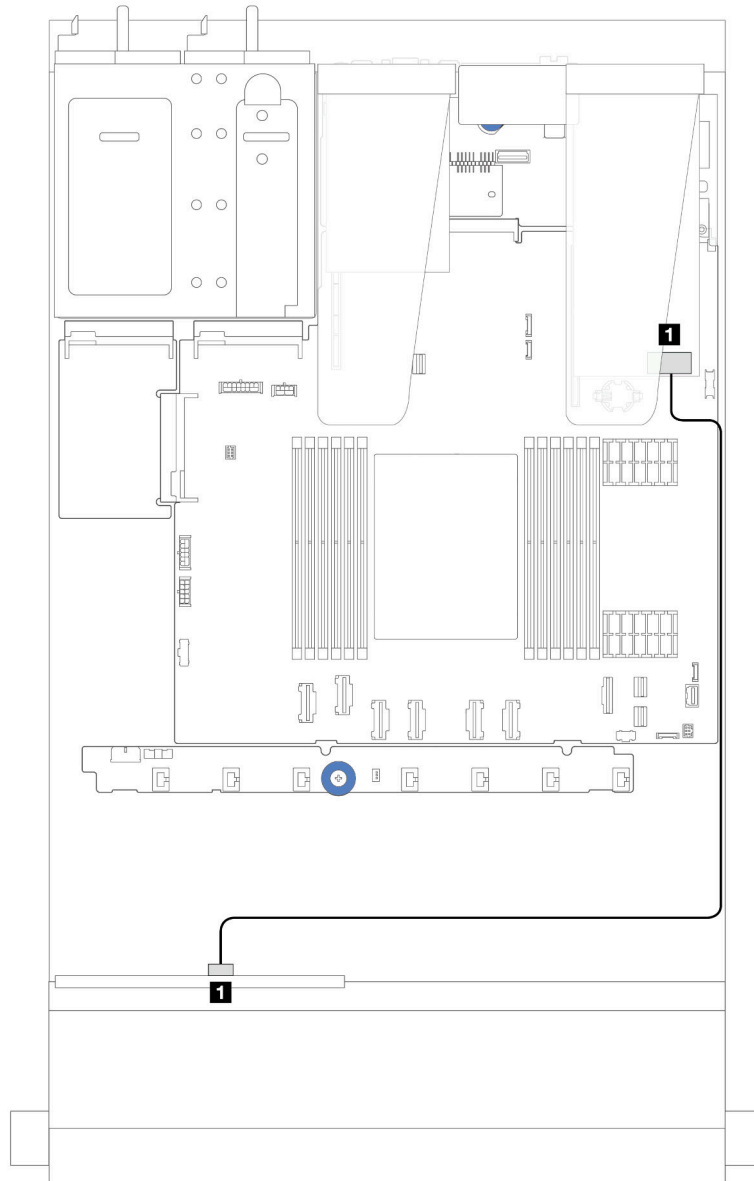
รูปภาพ 230. การเดินสายสำหรับช่องใส่ไดรฟ์ SAS/SATA ด้านหน้าขนาด 2.5 นิ้ว 4 ชุดที่มีอะแดปเตอร์ 8i SFF RAID (Gen 3/ Gen 4)
