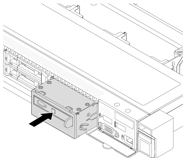
รูปภาพ 44. การติดตั้งส่วนประกอบแผงการวินิจฉัย
