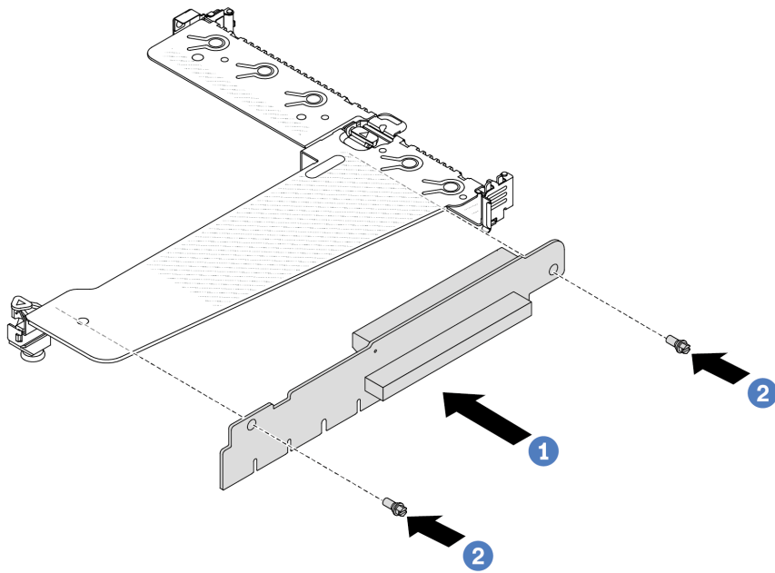
รูปภาพ 151. การติดตั้งการ์ด ตัวยก
