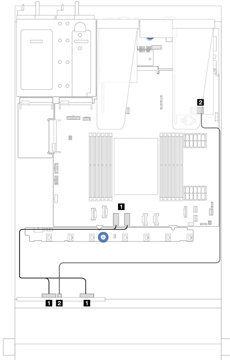
รูปภาพ 233. การเดินสายช่องใส่ไดรฟ์ NVMe ด้านหน้าขนาด 2.5 นิ้ว 4 ช่อง (โดยใช้แบ็คเพลน AnyBay ขนาด 2.5 นิ้ว 4 ชุด (Gen 5)) และอะแดปเตอร์ SFF 8i RAID/HBA (Gen 3/Gen 4)
