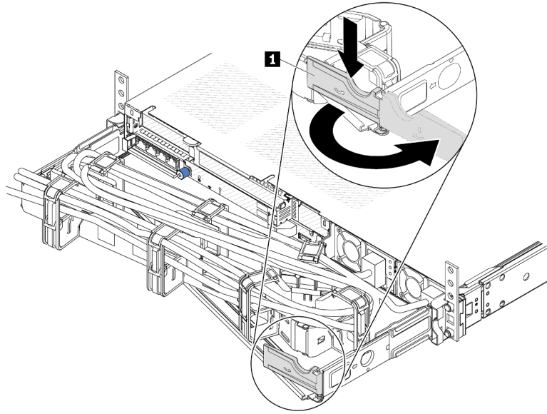
รูปภาพ 67. การปรับ CMA
