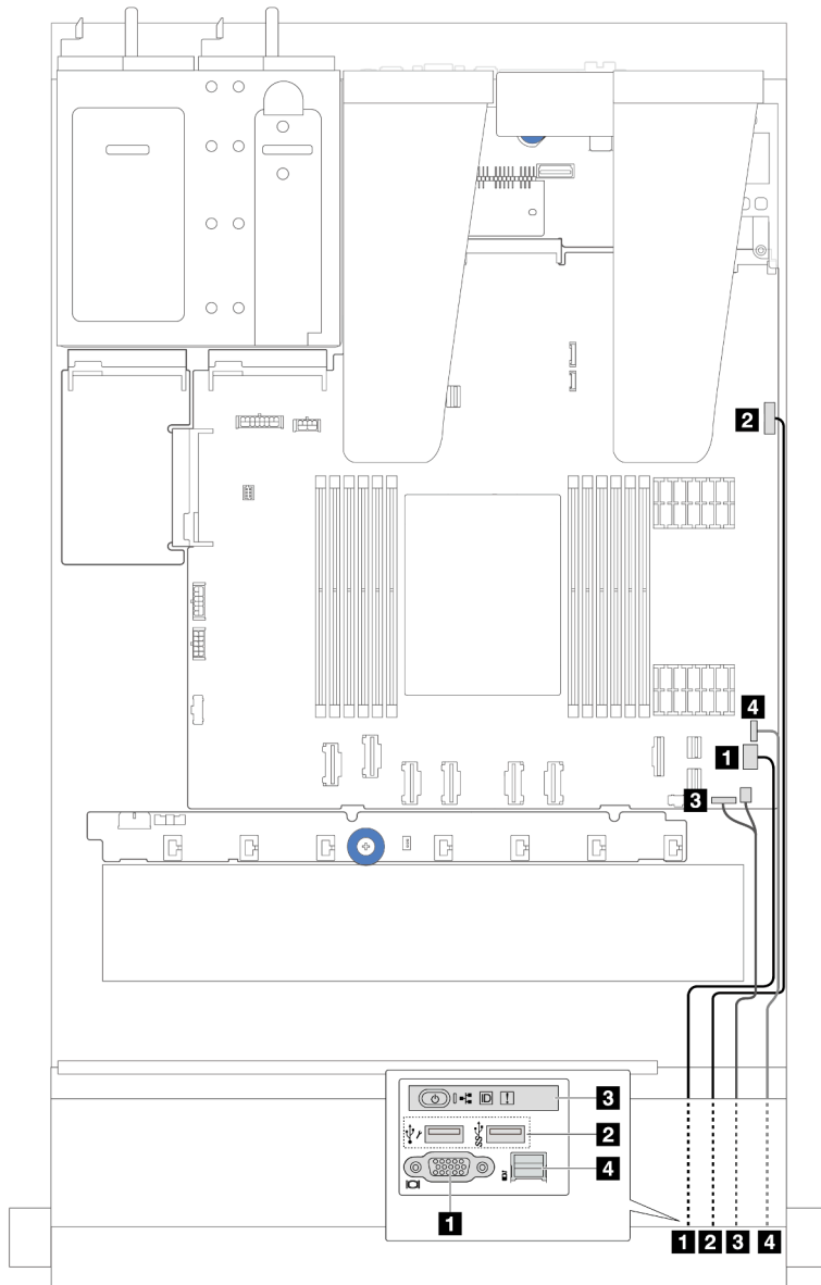
รูปภาพ 202. การเดินสายโมดูล I/O ด้านหน้าบนตัวเครื่องขนาด 2.5 นิ้ว
