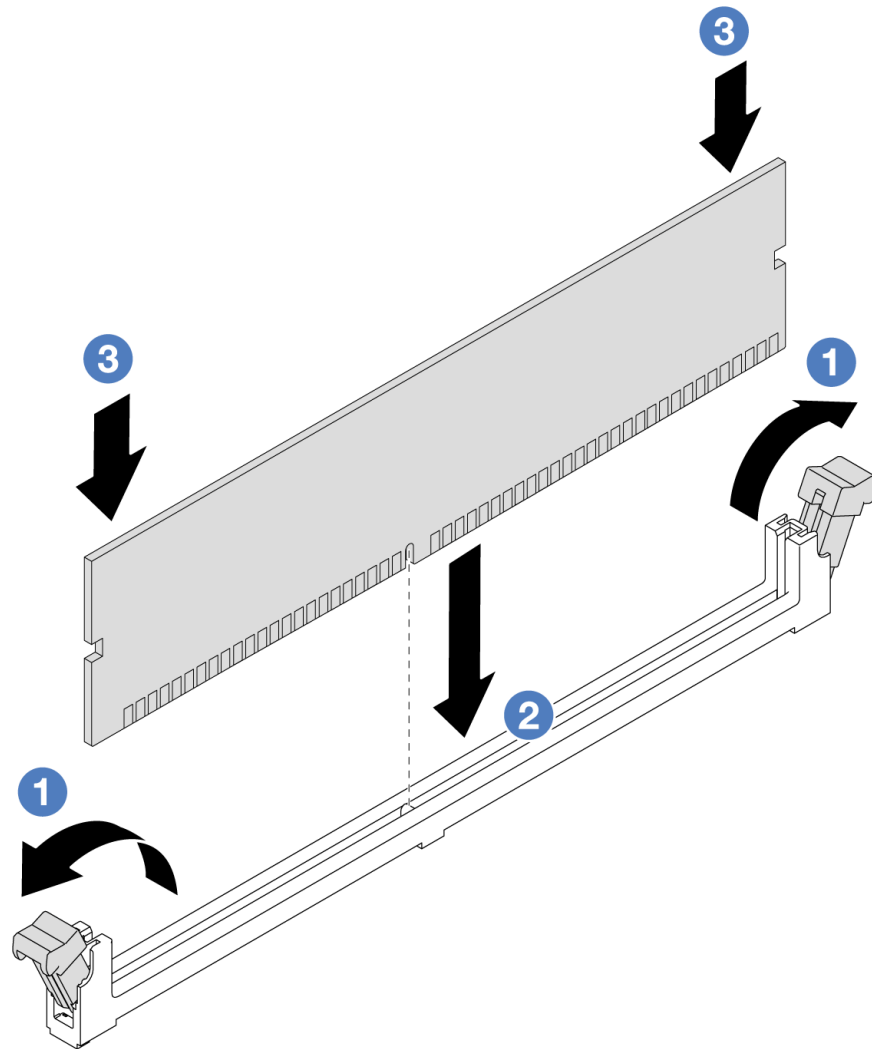
รูปภาพ 78. การติดตั้งโมดูลหน่วยความจำ
