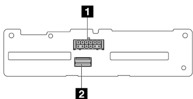
รูปภาพ 194. แบ็คเพลน SAS/SATA ขนาด 2.5 นิ้ว 4 ชุด
