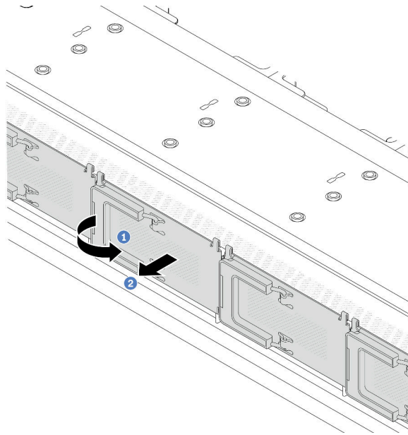
รูปภาพ 62. การถอดฝาครอบตัวครอบไดรฟ์ EDSFF
