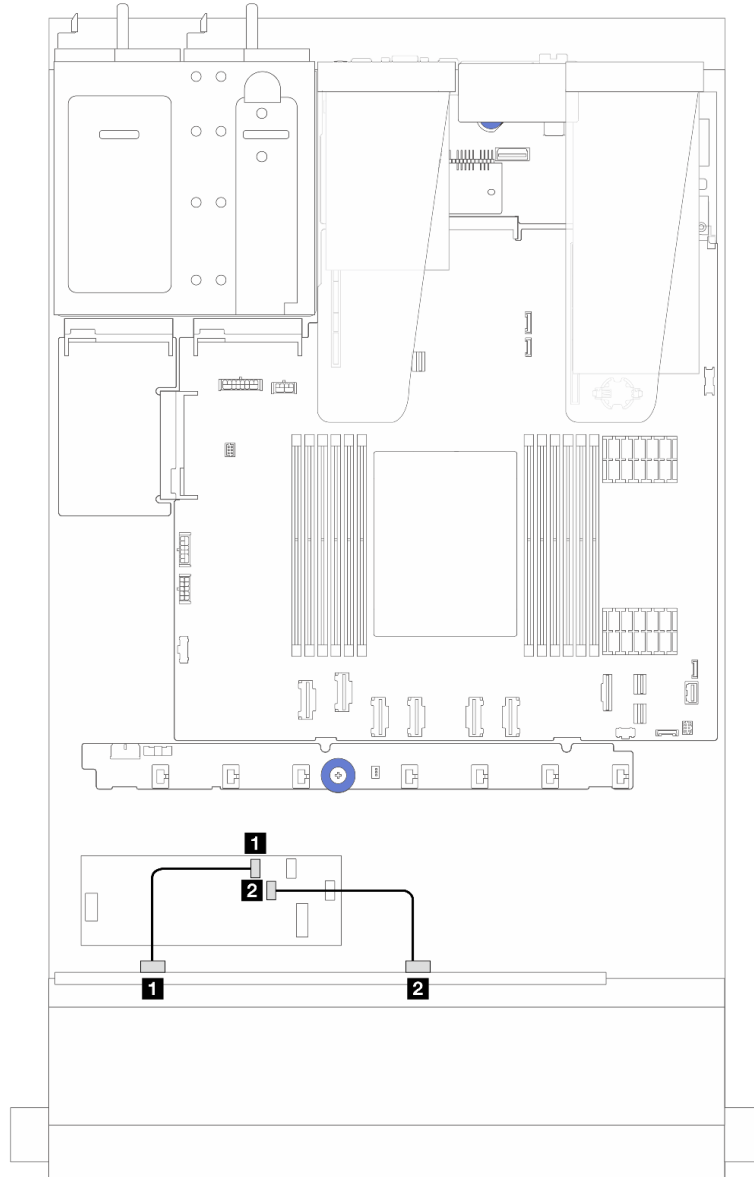
รูปภาพ 238. การเดินสายสำหรับช่องใส่ไดรฟ์ SAS/SATA ด้านหน้าขนาด 2.5 นิ้ว 8 ชุดที่มีอะแดปเตอร์ 16i CFF RAID/HBA (Gen 4)
