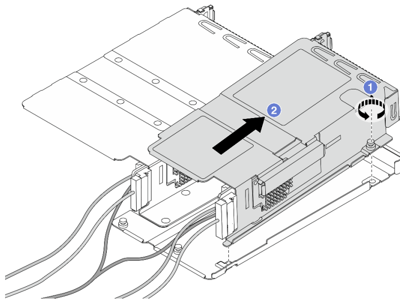
รูปภาพ 25. การแยกตัวครอบสองตัว
