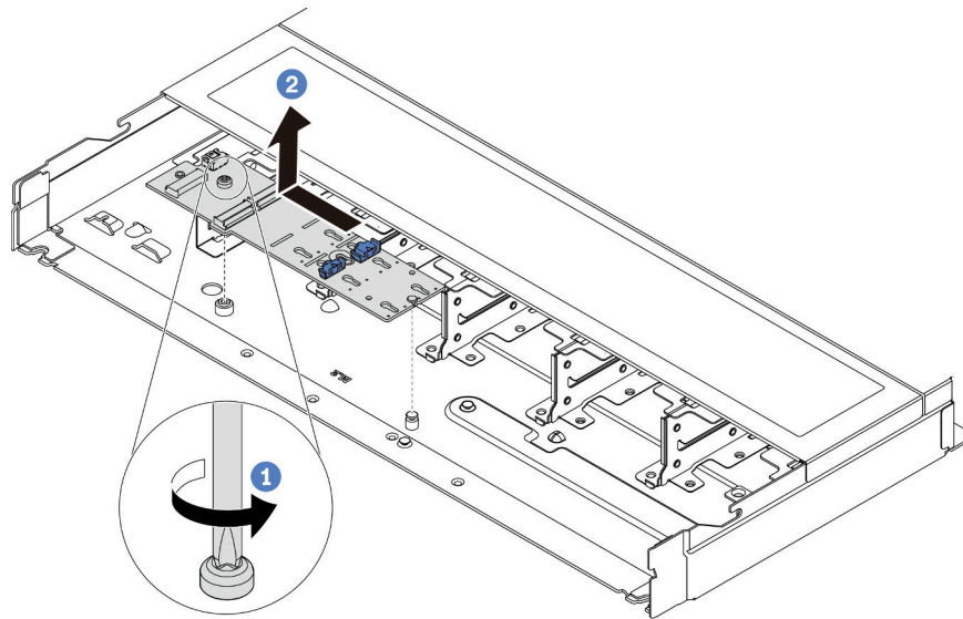
รูปภาพ 80. การถอดโมดูล M.2
