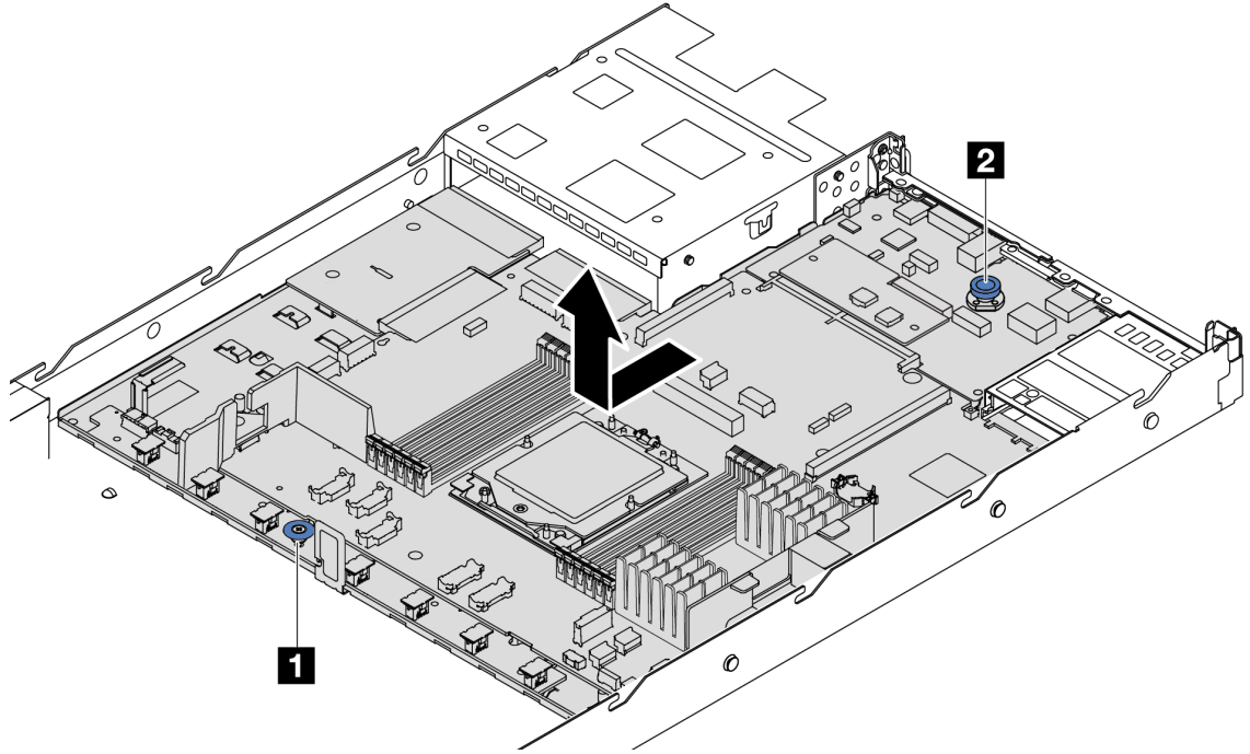
รูปภาพ 181. การถอดส่วนประกอบแผงระบบ
