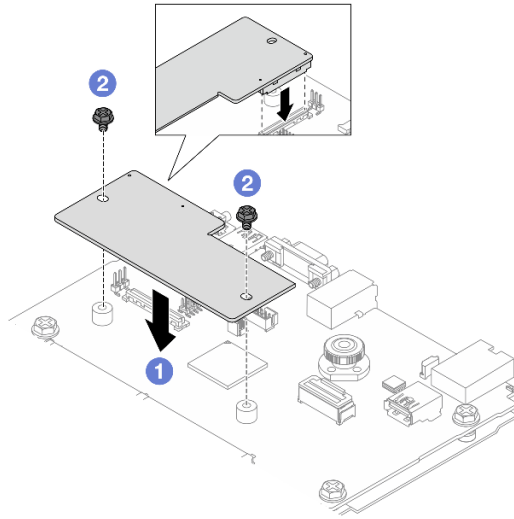
รูปภาพ 179. การติดตั้ง โมดูลนิรภัยของเฟิร์มแวร์และ RoT
