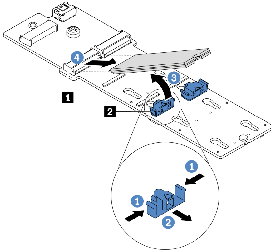
รูปภาพ 79. การถอดไดรฟ์ M.2
