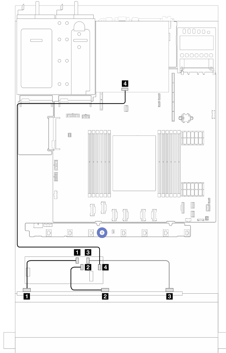
รูปภาพ 248. การเดินสายช่องใส่ไดรฟ์ SAS/SATA ด้านหน้า 6 ตัว และ AnyBay ด้านหน้า 4 ตัว และอะแดปเตอร์ CFF RAID 16i (Gen 3/Gen 4) ที่มีการติดตั้งไดรฟ์ SAS/SATA ด้านหลัง ขนาด 2.5 นิ้ว 2 ชุด
