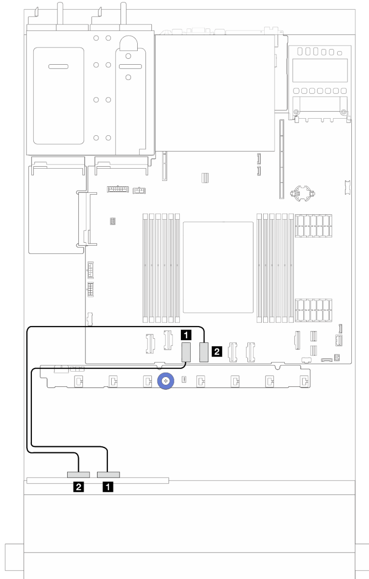
รูปภาพ 231. การเดินสายสำหรับการกำหนดค่าบนแผงของช่องใส่ไดรฟ์ NVMe ด้านหน้าขนาด 2.5 นิ้ว 4 ชุด (โดยใช้แบ็คเพลน AnyBay ขนาด 2.5 นิ้ว 4 ตัว (Gen 4))
