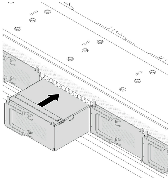
รูปภาพ 16. การติดตั้งตัวครอบ EDSFF
