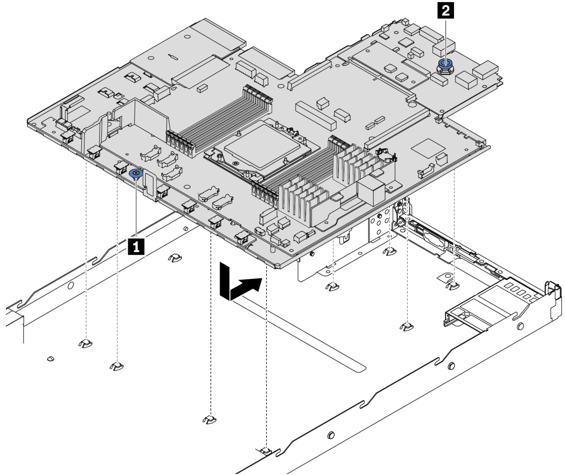
รูปภาพ 184. การติดตั้งส่วนประกอบแผงระบบ
