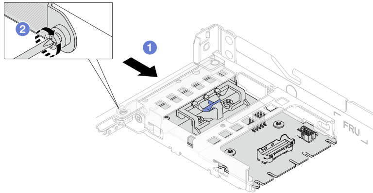
รูปภาพ 38. การติดตั้งอินเทอร์โพเซอร์ OCP ด้านหลัง
