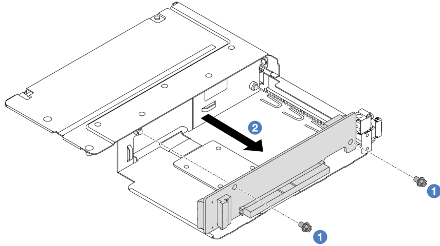
รูปภาพ 28. การถอดการ์ดด้วยก๊อกรอกจากตัวครอบแบบสูงเต็มที่
