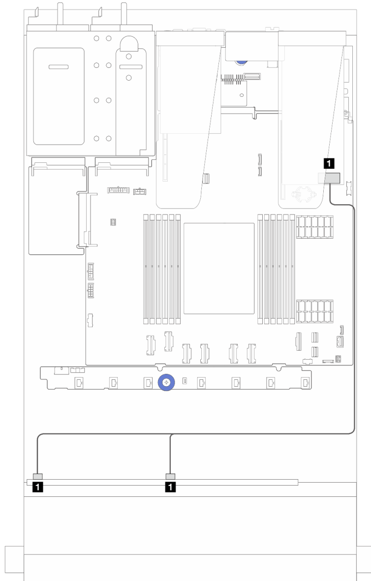
รูปภาพ 249. การเดินสายช่องใส่ไดรฟ์ SAS/SATA 6 ตัว และ AnyBay 2 ตัว และ NVMe ด้านหน้า 2 ตัว ที่มีอะแดปเตอร์ SFF RAID 8i (Gen 4)
