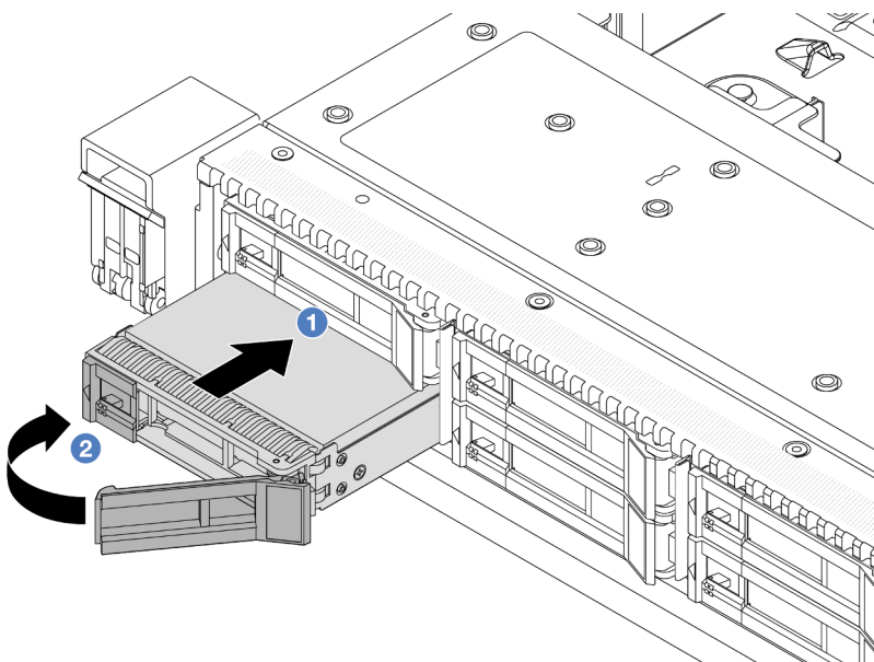
รูปภาพ 61. การติดตั้งไดรฟ์แบบ Hot-swap
