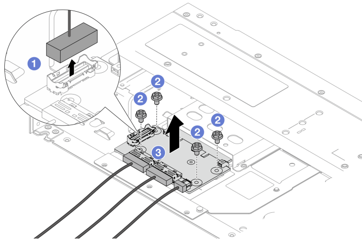
รูปภาพ 35. การถอดการ์ดอินเทอร์เฟซ OCP ด้านหน้า
