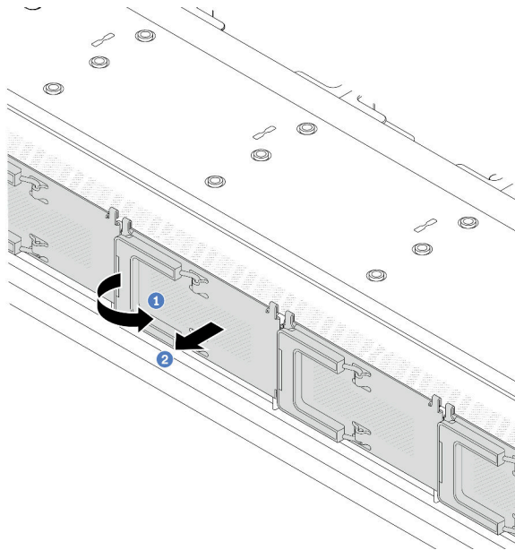
รูปภาพ 17. การถอดฝาครอบตัวครอบไดรฟ์ EDSFF
