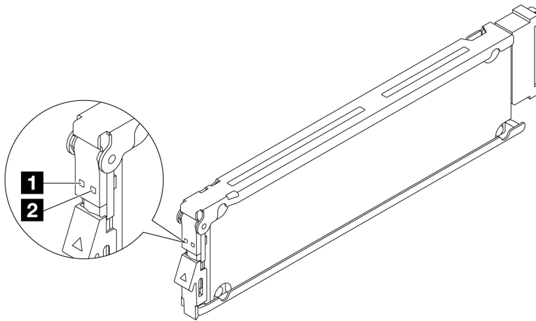
รูปภาพ 256. ไฟ LED บนไดรฟ์ EDSFF
