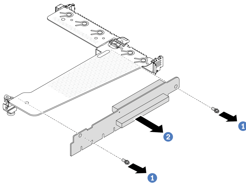
รูปภาพ 149. การถอดการ์ด ตัวยก
