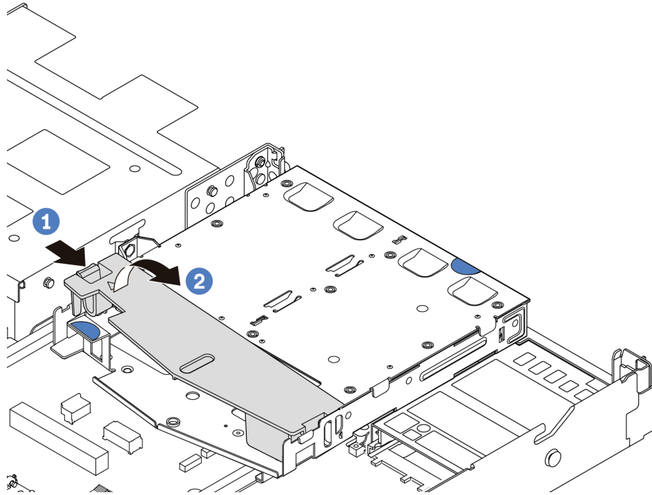
รูปภาพ 159. การถอดแผ่นกั้นลม
