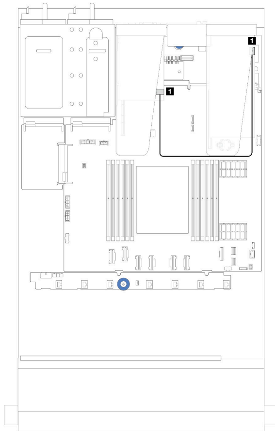
รูปภาพ 209. การเดินสายของโมดูลพลังงานแบบแฟลชของ RAID บนส่วนประกอบตัวแยก
