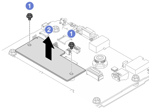
รูปภาพ 178. การถอด โมดูลนิรภัยของเฟิร์มแวร์และ RoT
