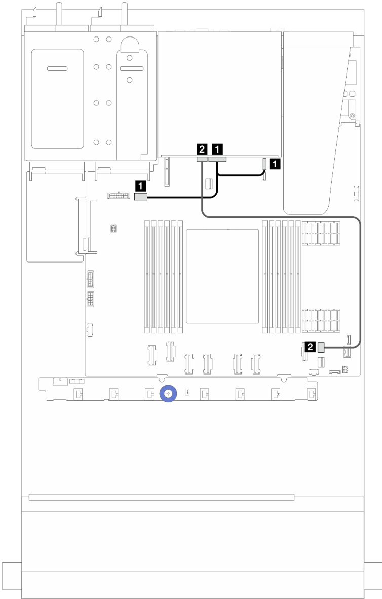
รูปภาพ 213. การเดินสายแบ็คเพลนไดรฟ์ SATA ด้านหลัง ขนาด 2.5 นิ้ว 2 ชุด
