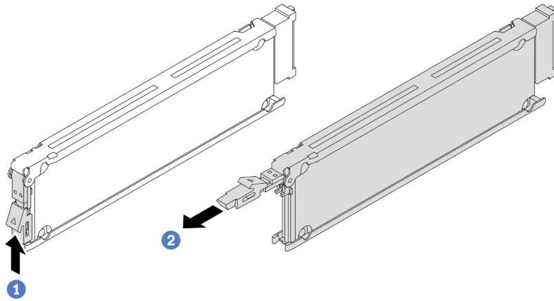
รูปภาพ 63. การถอดไดรฟ์ EDSFF
