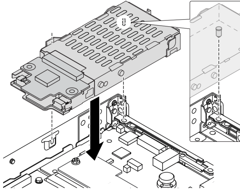
รูปภาพ 165. การติดตั้งตัวครอบไดรฟ์ด้านหลังแบบ Hot-swap
