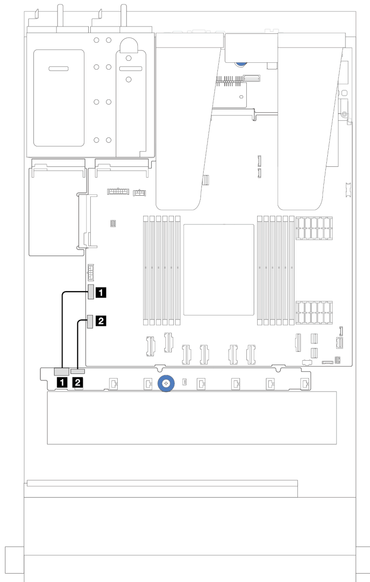
รูปภาพ 228. การเดินสาย Sideband และสายไฟแผงพัดลม
