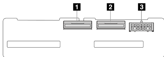
รูปภาพ 195. แบ็คเพลน NVMe ขนาด 2.5 นิ้ว 4 ชุด
