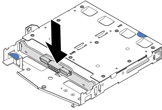
รูปภาพ 160. การติดตั้งแบ็คเพลนด้านหลัง
