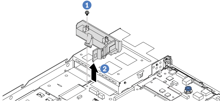
รูปภาพ 89. การถอดแผ่นกั้นลมชุดแหล่งจ่ายไฟ
