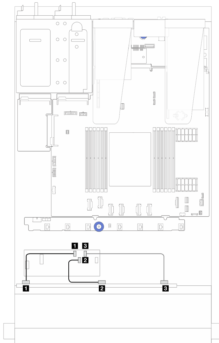
รูปภาพ 246. การเดินสายช่องใส่ไดรฟ์ SAS/SATA ด้านหน้า 6 ตัว และ AnyBay ด้านหน้า 4 ตัว และอะแดปเตอร์ 16i CFF RAID/HBA (Gen 3)
