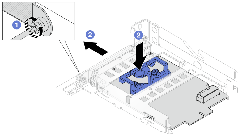
รูปภาพ 75. การถอดอะแดปเตอร์ NIC การจัดการ
