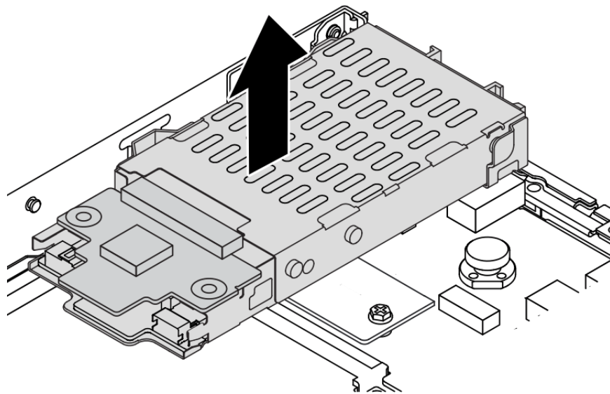
รูปภาพ 164. การถอดตัวครอบไดรฟ์ด้านหลังแบบ Hot-swap
