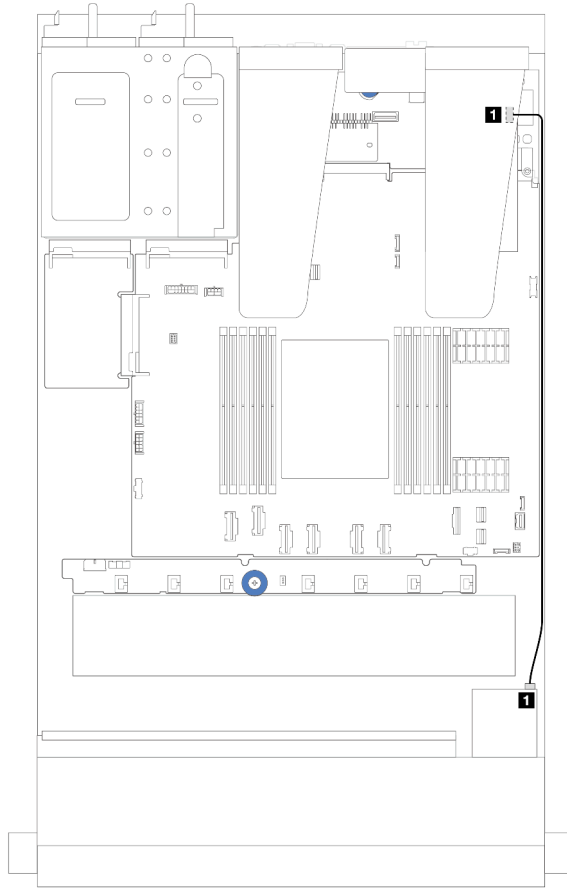
รูปภาพ 207. การเดินสายโมดูลพลังงานแบบแฟลชของ RAID สำหรับอะแดปเตอร์ SFF RAID/HBA
