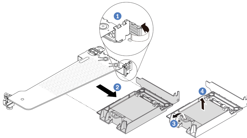
รูปภาพ 114. การถอดโมดูลพลังงานแบบแฟลชของ RAID ออกจากส่วนประกอบตัวยก
