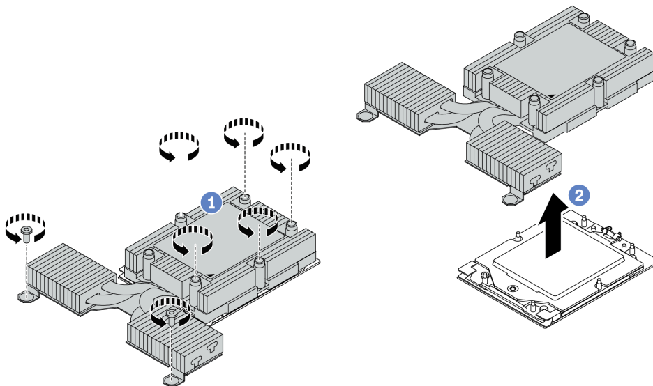
รูปภาพ 92. การถอดตัวระบายความร้อนที่ระบายความร้อนด้วยอากาศ
