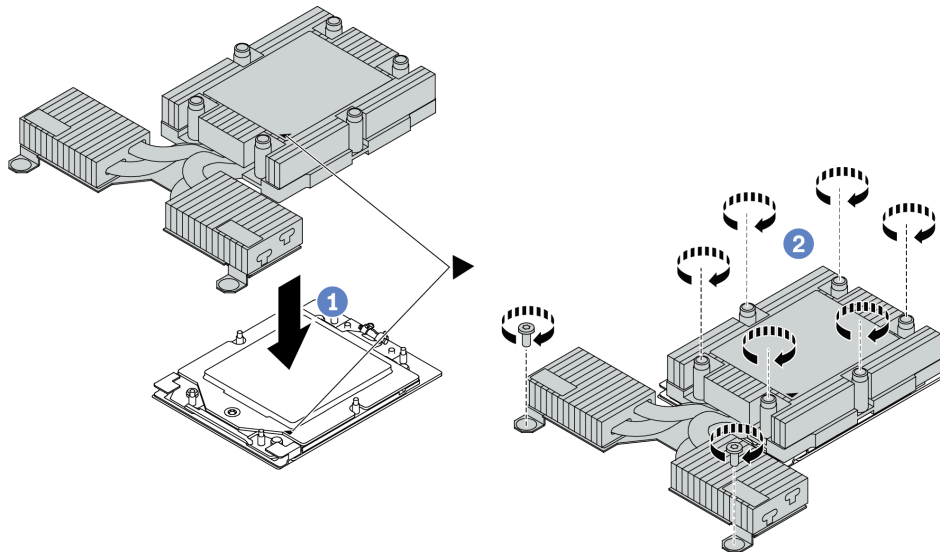
รูปภาพ 95. การติดตั้งตัวระบายความร้อนที่ระบายความร้อนด้วยอากาศ
