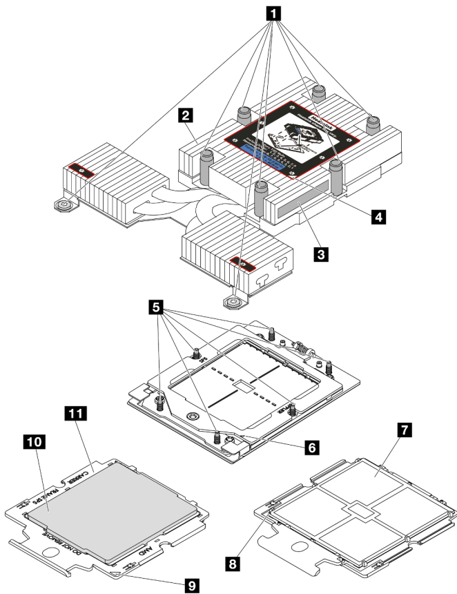
รูปภาพ 91. ส่วนประกอบโปรเซสเซอร์และตัวระบายความร้อน
