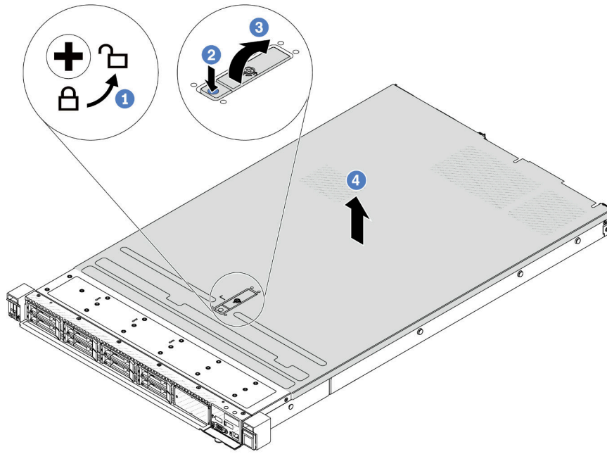
รูปภาพ 187. การถอดฝาครอบด้านบน
