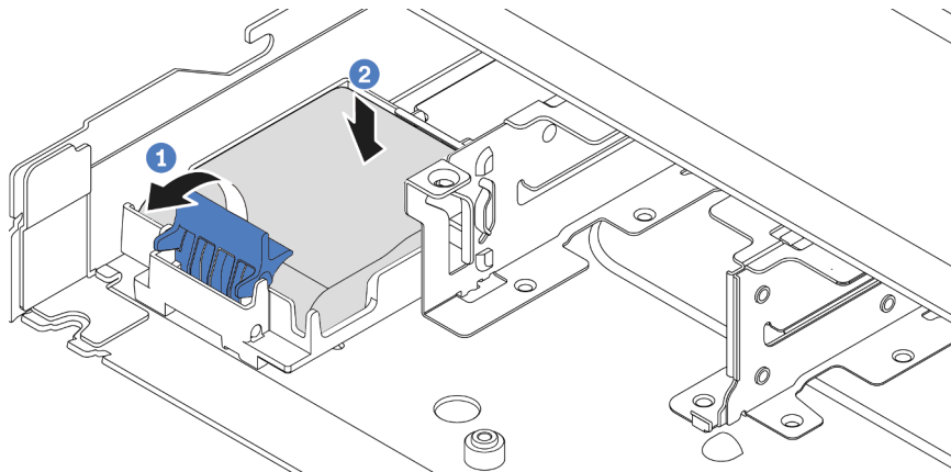
รูปภาพ 113. การติดตั้งโมดูลพลังงานแบบแฟลชของ RAID บนถาดแผงระบบ
