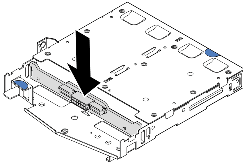
รูปภาพ 7. การติดตั้งแบ็คเพลนด้านหลัง
