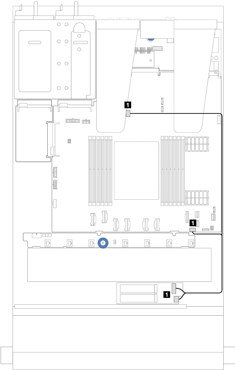
รูปภาพ 222. การเดินสายสำหรับ ThinkSystem M.2 NVMe 2-Bay RAID Enablement Kit
