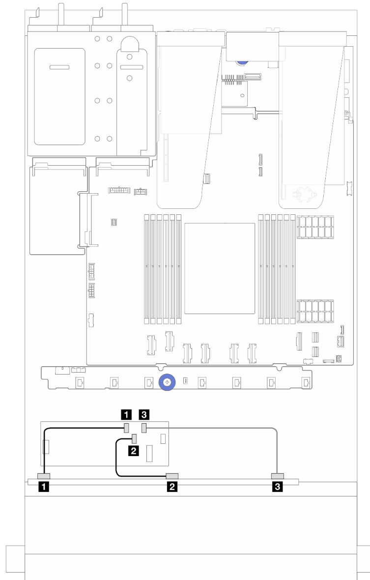
รูปภาพ 247. การเดินสายช่องใส่ไดรฟ์ SAS/SATA ด้านหน้า 6 ตัว และ AnyBay ด้านหน้า 4 ตัว และอะแดปเตอร์ CFF RAID 16i (Gen 3 หรือ Gen 4)
