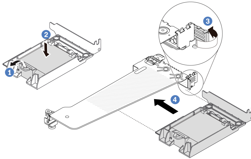
รูปภาพ 115. การติดตั้งโมดูลพลังงานแบบแฟลชของ RAID บนส่วนประกอบตัวยก
