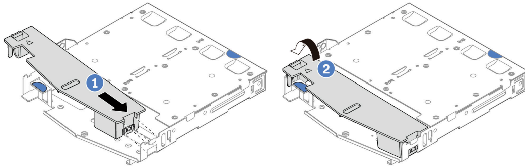
รูปภาพ 161. การติดตั้งแผ่นกันลม
