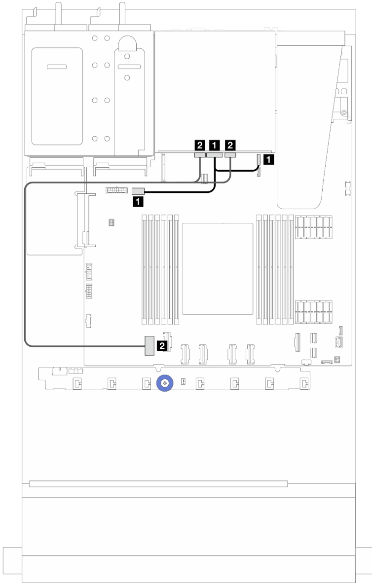
รูปภาพ 212. การเดินสายแบ็คเพลนไดรฟ์ NVMe ด้านหลัง ขนาด 2.5 นิ้ว 2 ช่อง
