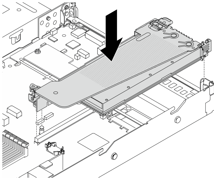
รูปภาพ 50. การติดตั้งส่วนประกอบด้วยก
