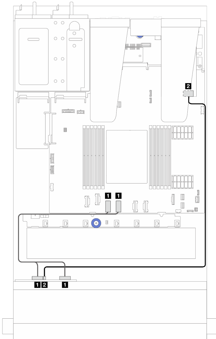
รูปภาพ 234. การเดินสายสำหรับแบ็คเพลนไดรฟ์ AnyBay ขนาด 2.5 นิ้ว 4 ตัว พร้อมอะแดปเตอร์ 8i SFF RAID (Gen 3 หรือ Gen 4)
