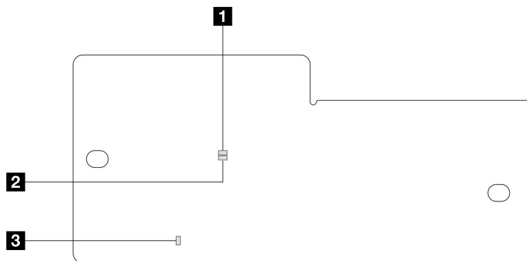
图 22. 固件和 RoT 安全模块上的 LED
