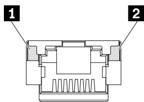
图 21. XCC 系统管理端口 LED
