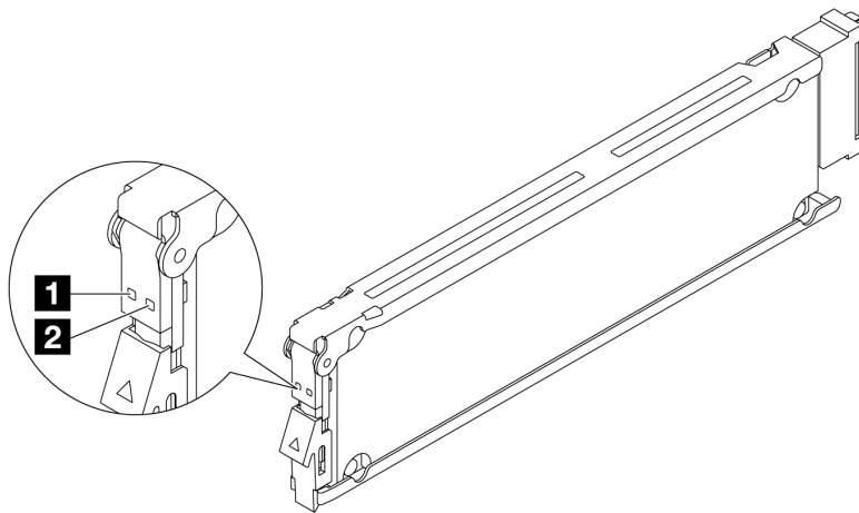
图 17. EDSFF 硬盘上的 LED
