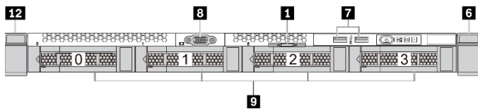
Abbildung 3. Servermodelle mit vier 3,5-Zoll-Laufwerkpositionen
