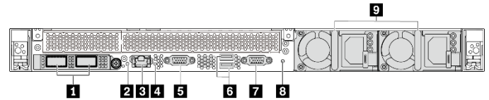
Abbildung 4. Servermodelle ohne PCIe-Steckplatz
