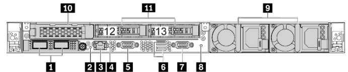
Abbildung 6. Servermodelle mit einem PCIe-Steckplatz und zwei 2,5-Zoll-Laufwerkpositionen an der Rückseite
