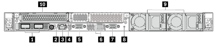
Abbildung 5. Servermodelle mit einem PCIe-Steckplatz
