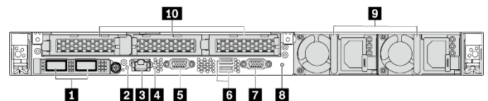
Abbildung 8. Servermodelle mit drei PCIe-Steckplätzen
