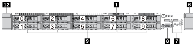
Abbildung 2. Servermodelle mit vier 2,5-Zoll-Laufwerkpositionen
