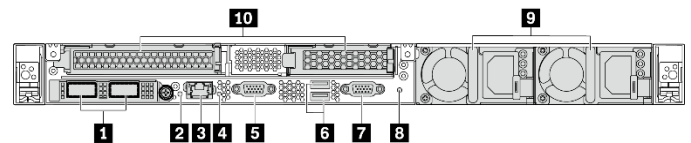
Abbildung 7. Servermodelle mit zwei PCIe-Steckplätzen
