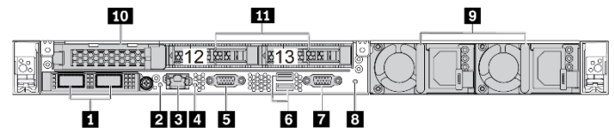
Figure 6. Modèles de serveur équipés d'un emplacement PCIe et de deux unités arrière 2,5 pouces
