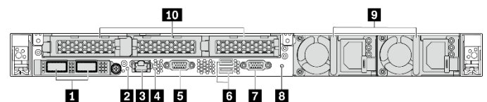
Figure 8. Modèles de serveur avec trois emplacements PCIe
