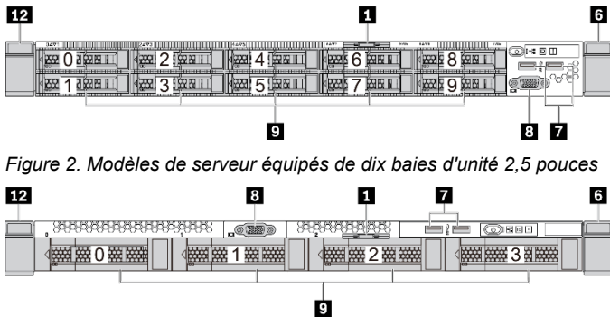
Figure 3. Modèles de serveur équipés de quatre baies d'unité 3,5 pouces
