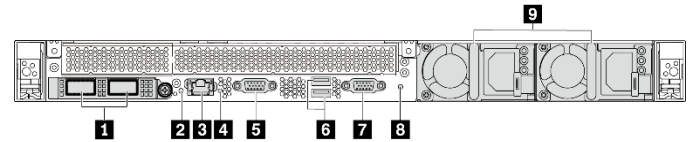
Figure 4. Modèles de serveur sans emplacement PCIe
