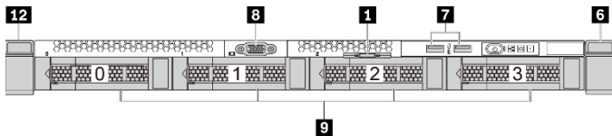
Figure 3. Modèles de serveur équipés de quatre baies d'unité 3,5 pouces
