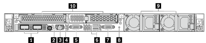
Figure 7. Modèles de serveur avec deux emplacements PCIe
