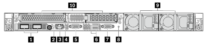
Figura 7. Modelos de servidor com dois slots PCIe
