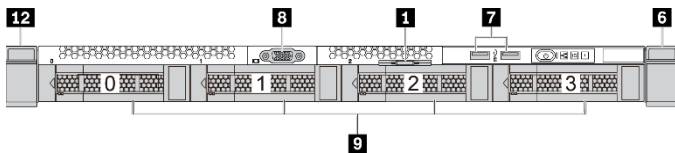
Figura 3. Modelos de servidor com quatro compartimentos de unidade de 3,5 polegadas
