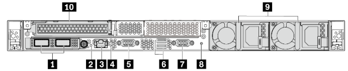
Figura 5. Modelos de servidor com um slot PCIe
