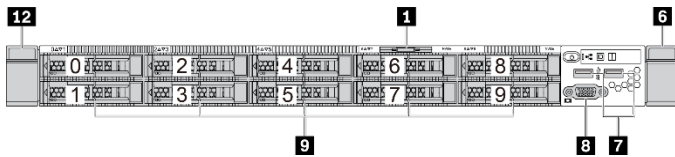
Figura 2. Modelos de servidor com dez compartimentos de unidade de 2,5 polegadas
