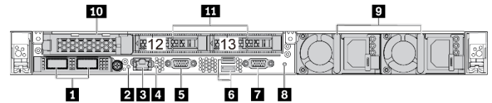
Figura 6. Modelos de servidor com um slot PCIe e dois compartimentos traseiros de unidade de 2,5 polegadas
