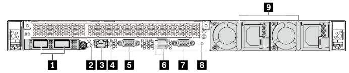
Figura 4. Modelos de servidor sem slots PCIe
