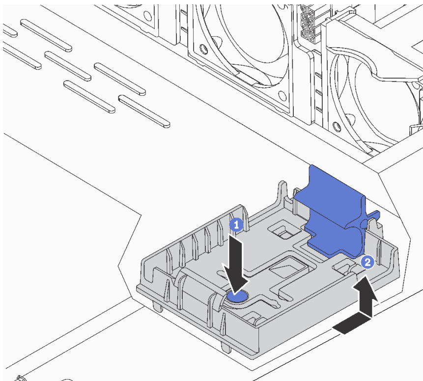
图 157. 卸下 RAID 超级电容器模块夹持器
