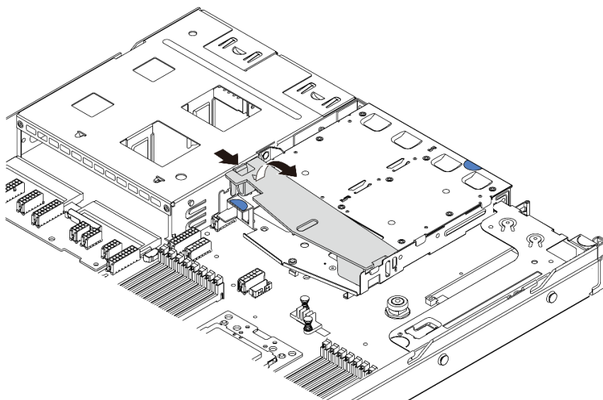
图 119. 卸下导风罩
