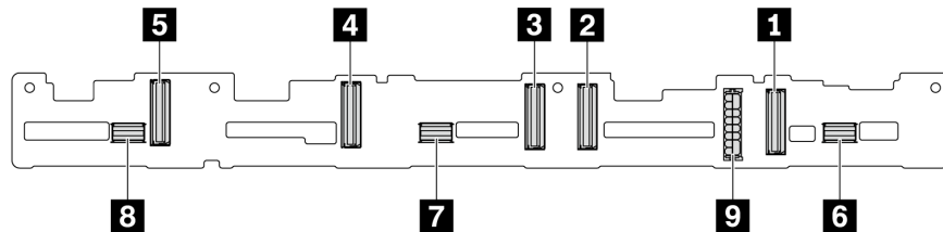
图 47. 用于十个 2.5 英寸 SAS/SATA/NVMe 硬盘的背板上的接口
