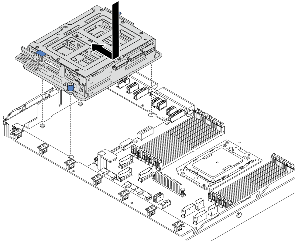
图 142. 安装中间硬盘仓 - 1
