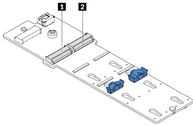
图 150. M.2 硬盘插槽
