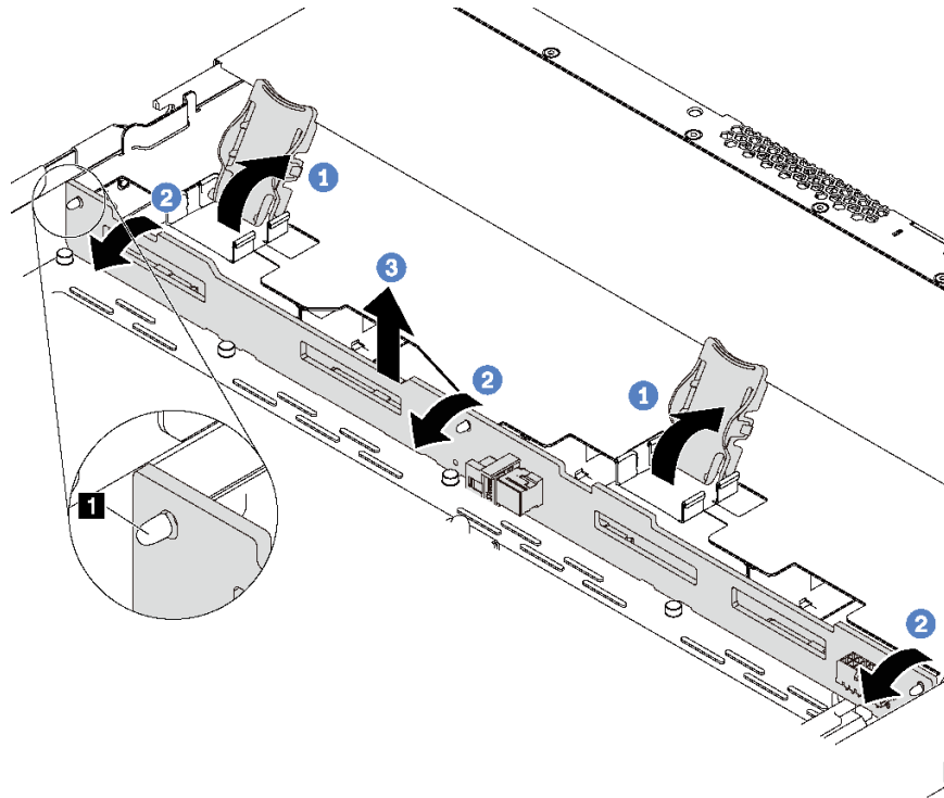
图 113. 卸下 4 x 3.5 英寸热插拔硬盘背板
