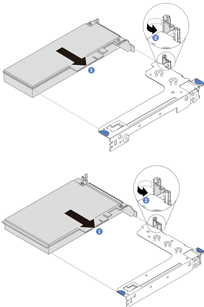
图 108. 安装转接卡 1 组合件 (LP/FHFL)
