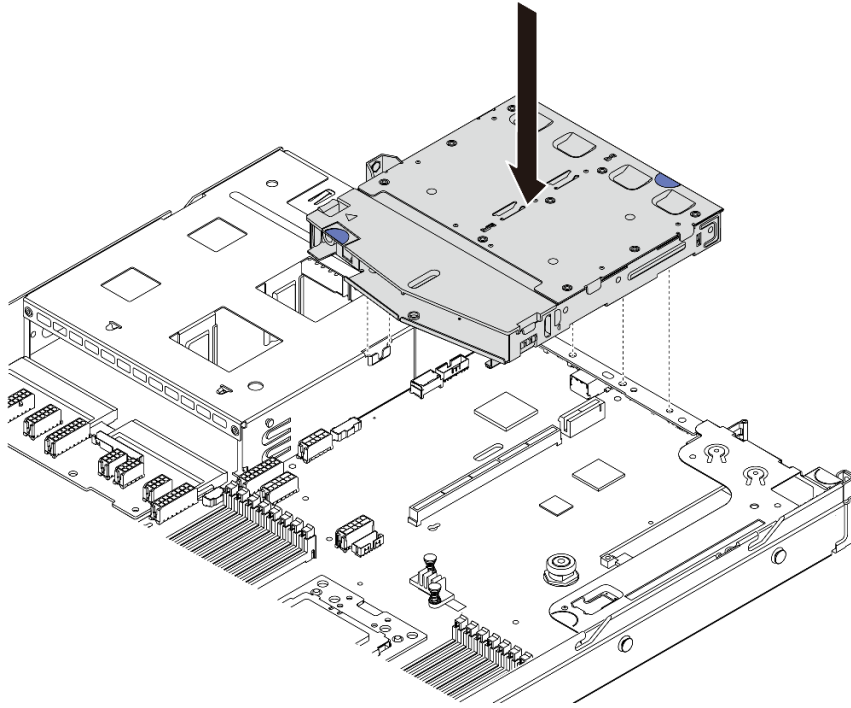
图 135. 安装背面热插拔硬盘仓
