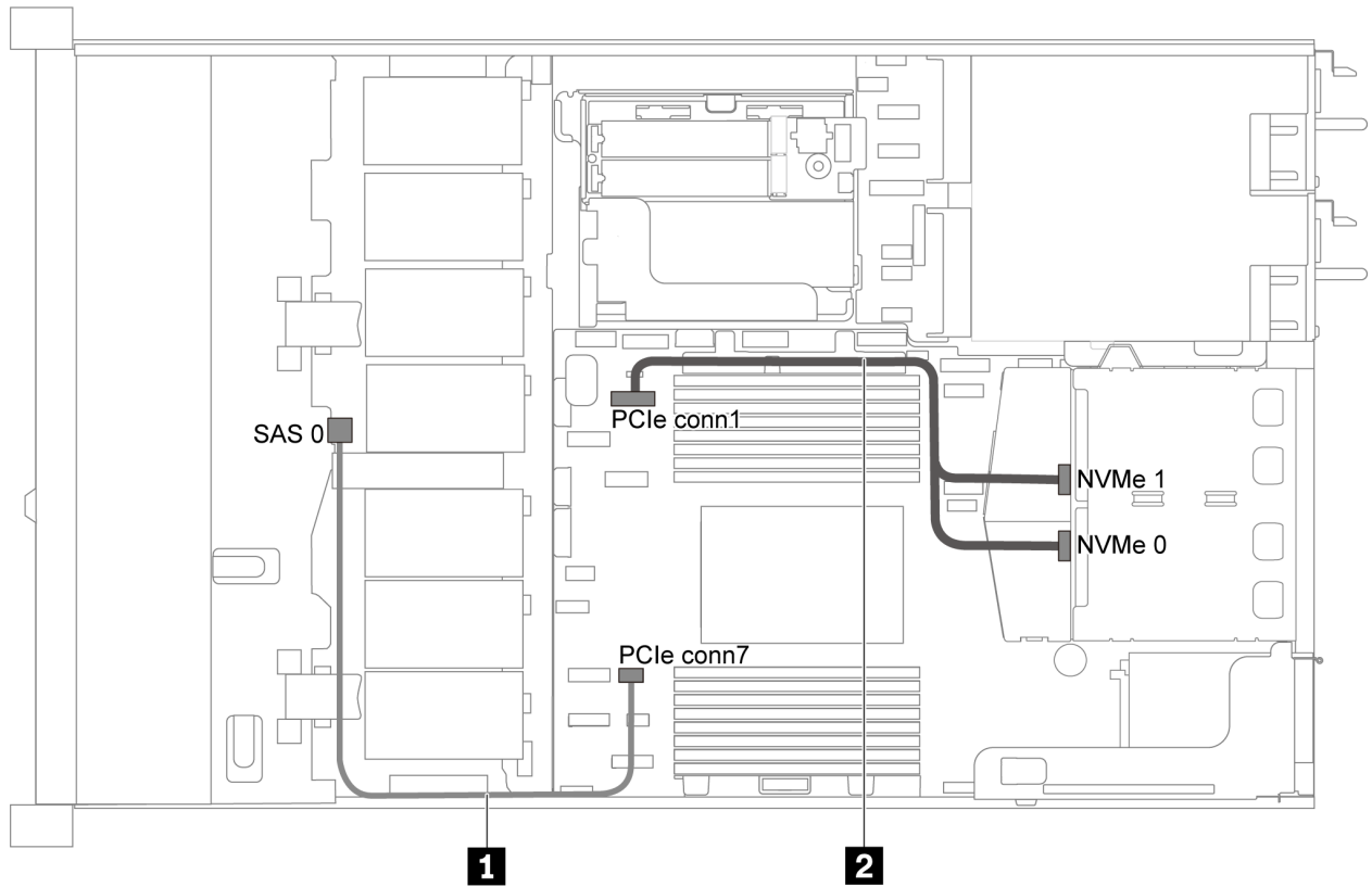
图 28. 配备四个 3.5 英寸 SATA 硬盘和背面 NVMe 硬盘组合件的服务器型号的线缆布放
