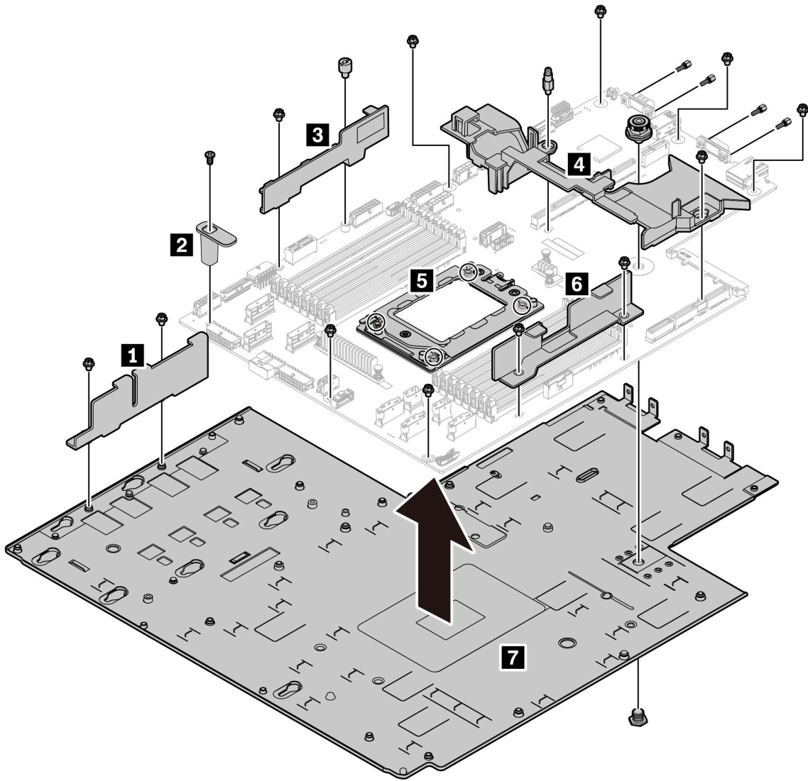
图 185. 拆卸主板
