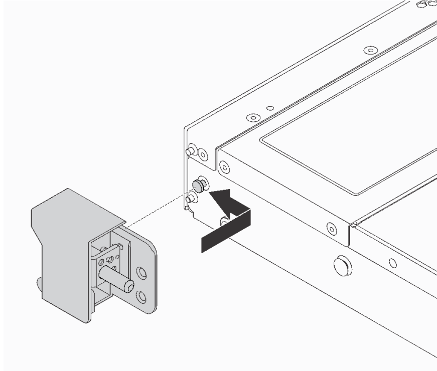
图 75. 安装机架滑锁
