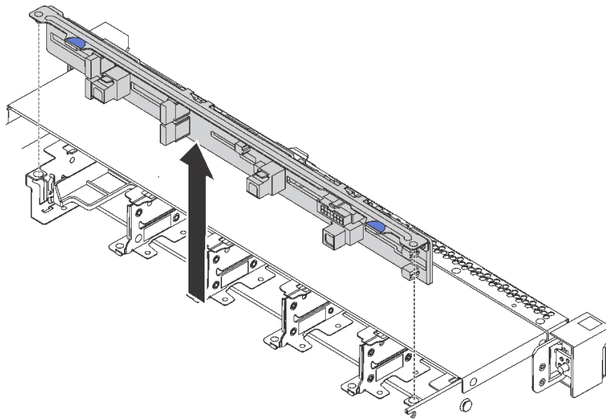
图 117. 卸下用于十个 2.5 英寸热插拔硬盘的背板
