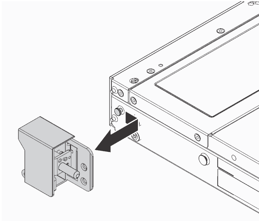
图 74. 卸下机架滑锁
