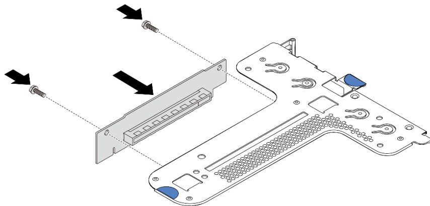
图 102. 安装转接卡
