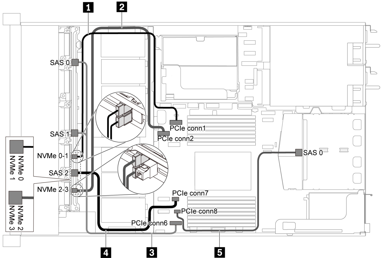
图 43. 配备六个 2.5 英寸 SATA 硬盘、四个 2.5 英寸 NVMe 硬盘和背面 SAS/SATA 硬盘组合件的服务器型号的线缆布放
