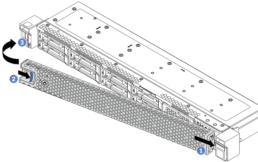
图 81. 安装安全挡板
