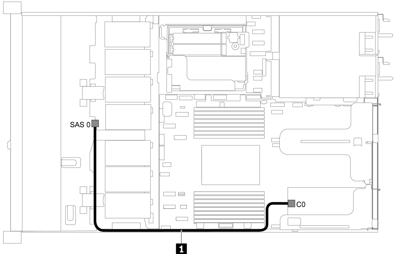
图 25. 配备四个 3.5 英寸 SAS/SATA 硬盘和一个 8i RAID/HBA 适配器的服务器型号的线缆布放
