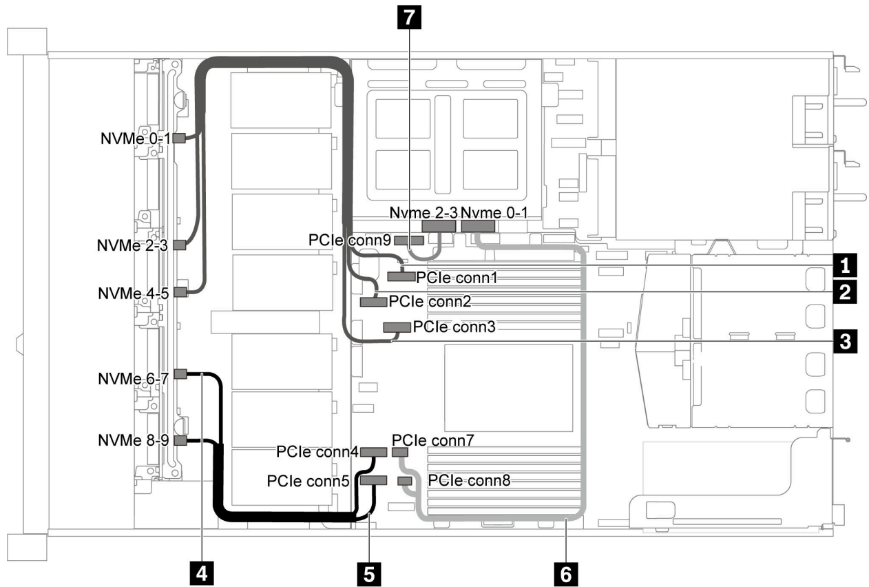
图 53. 配备十个 2.5 英寸 SAS/SATA/NVMe 硬盘、背面 SAS/SATA 硬盘组合件、中间 NVMe 硬盘组合件和一个 16i RAID/HBA 适配器的服务器型号的线缆布放 - 1
