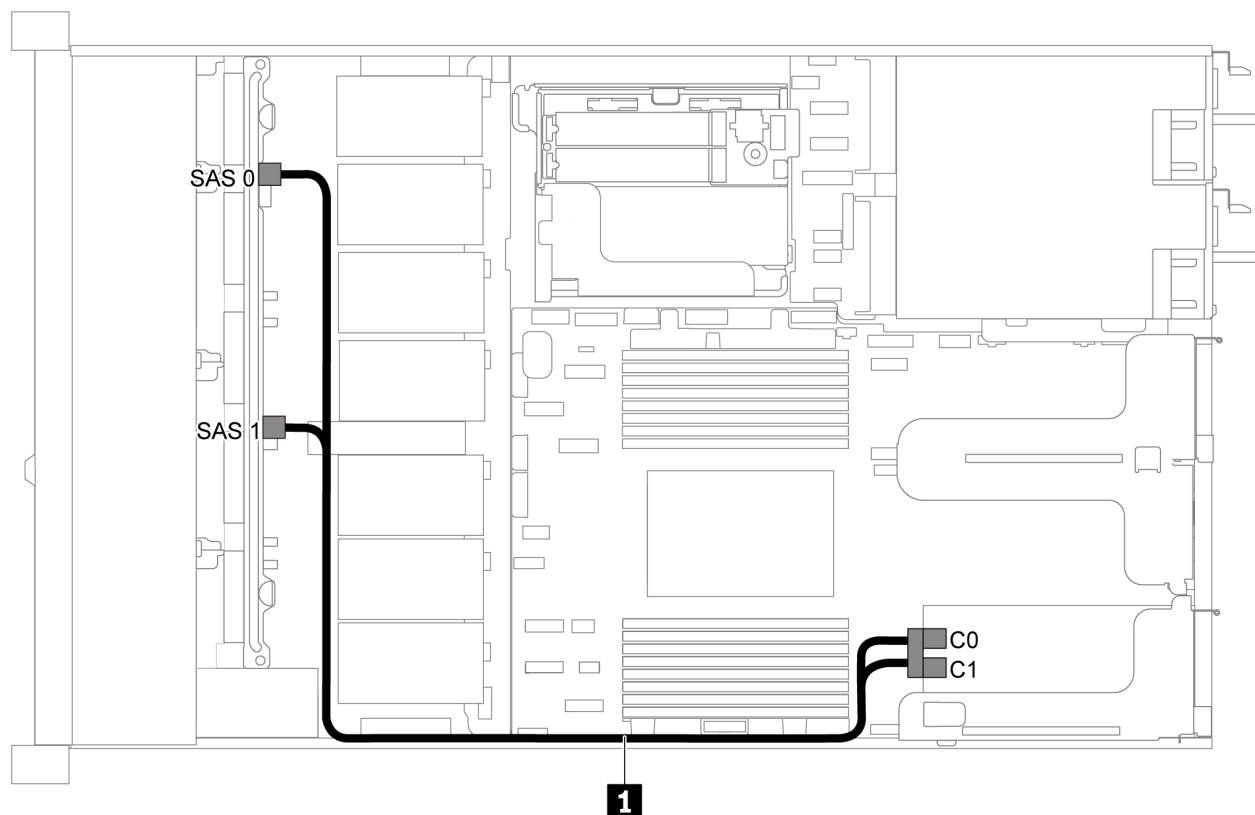
图 34. 配备八个 2.5 英寸 SAS/SATA 硬盘和一个 8i RAID/HBA 适配器的服务器型号的线缆布放
