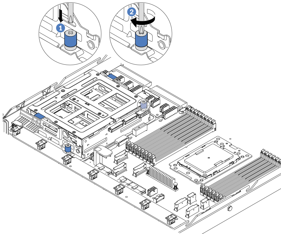
图 143. 安装中间硬盘仓 - 2
