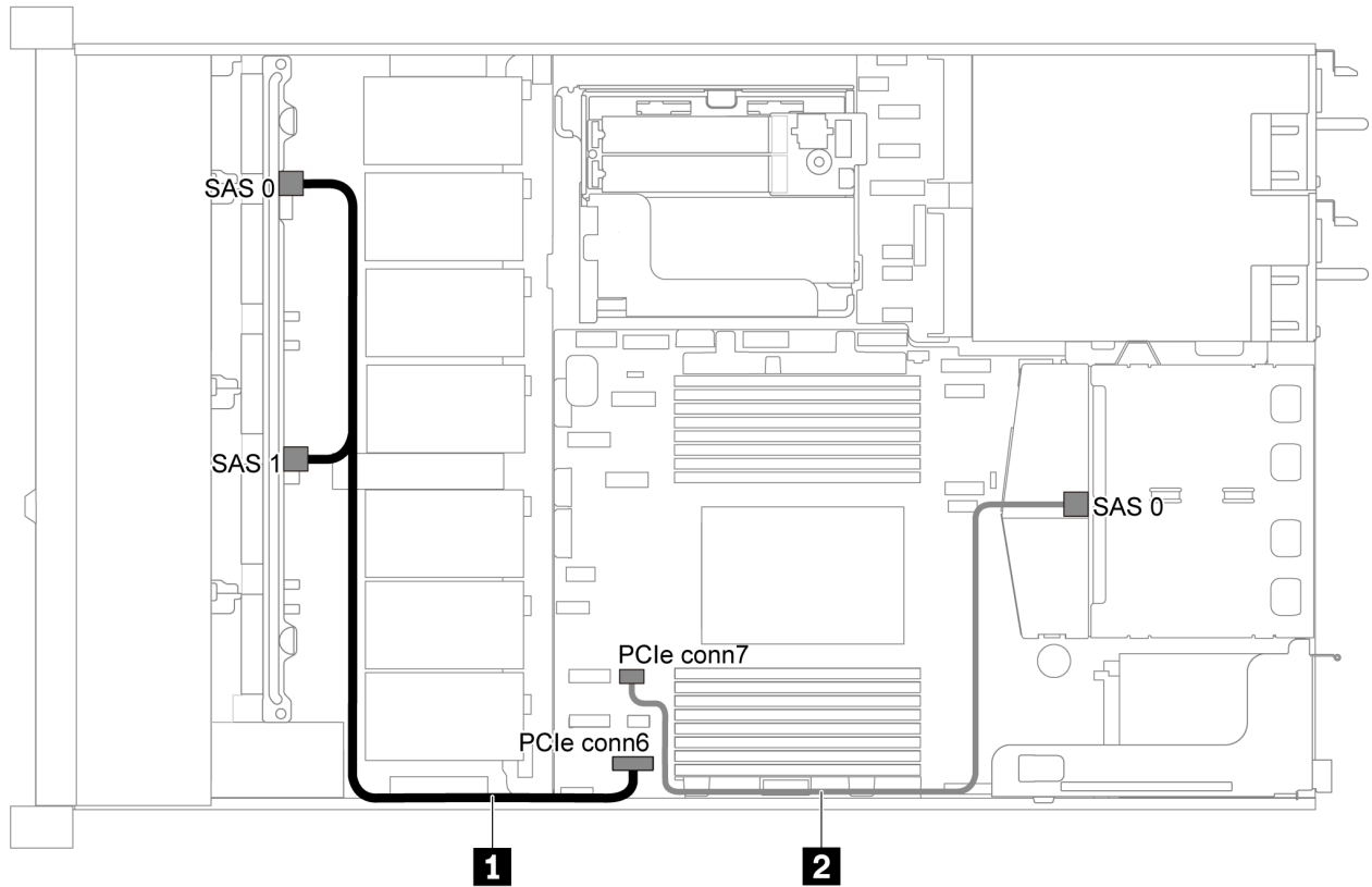
图 35. 配备八个 2.5 英寸 SATA 硬盘和背面 SAS/SATA 硬盘组合件的服务器型号的线缆布放
