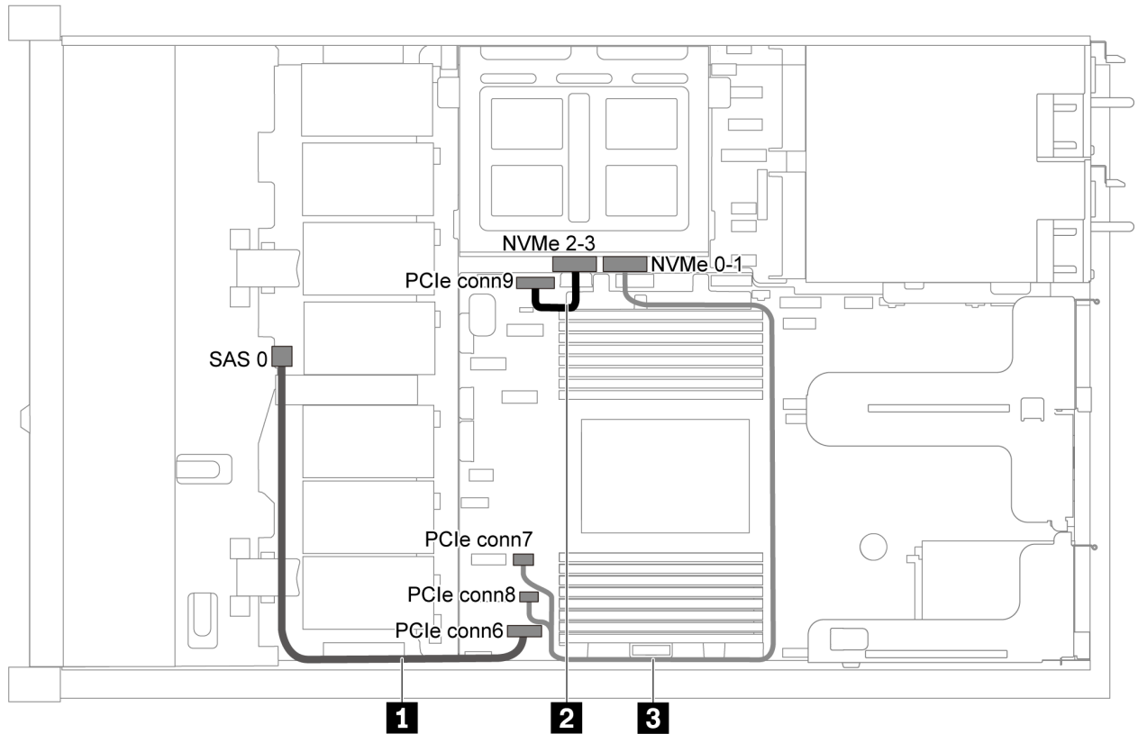
图 30. 配备四个 3.5 英寸 SATA 硬盘和中间硬盘仓的服务器型号的线缆布放
