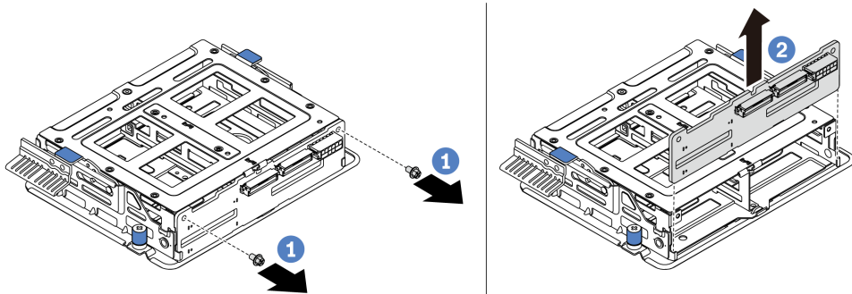
图 140. 卸下内部背板
