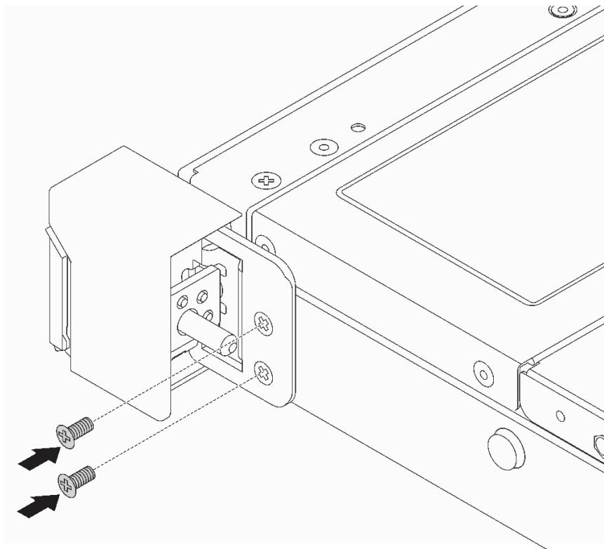
图 76. 安装机架滑锁螺钉
