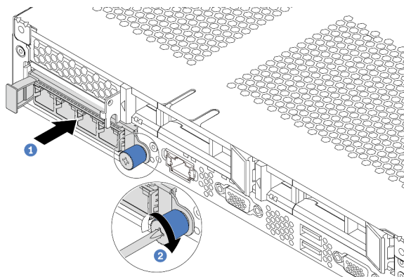
图 92. 安装 OCP 3.0 以太网适配器
