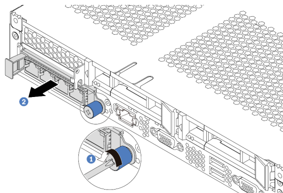
图 91. 卸下 OCP 3.0 以太网适配器
