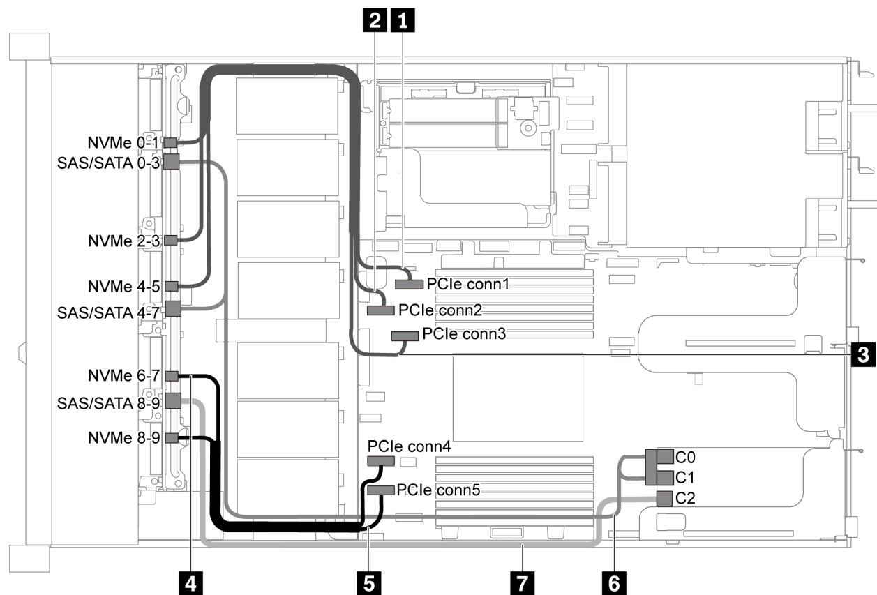
图 49. 配备十个 2.5 英寸 SAS/SATA/NVMe 硬盘和一个 16i RAID/HBA 适配器的服务器型号的线缆布放
