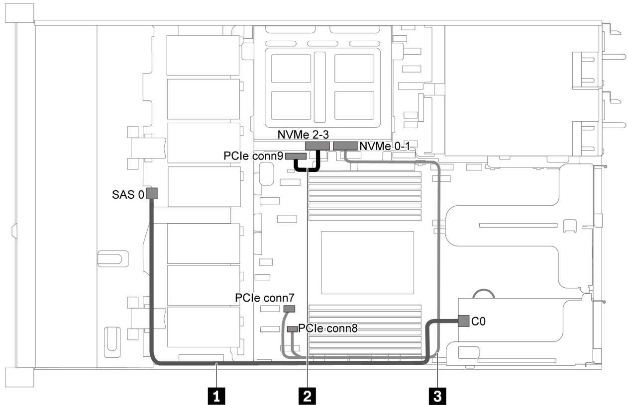
图 31. 配备四个 3.5 英寸 SAS/SATA 硬盘、中间硬盘仓和一个 8i RAID/HBA 适配器的服务器型号的线缆布放
