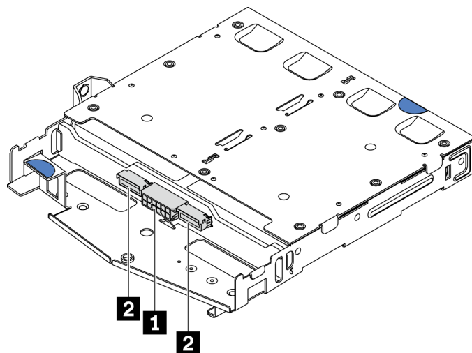
图 122. NVMe 背面背板接口
