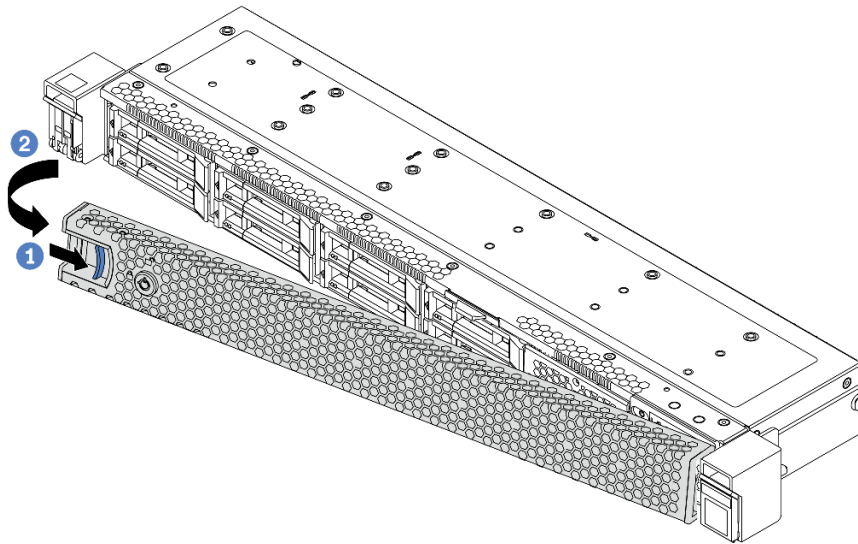
图 79. 卸下安全挡板
