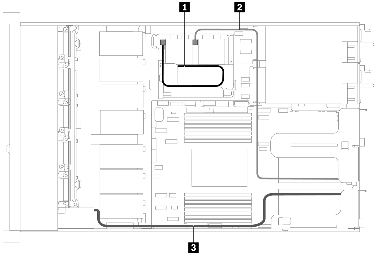
图 62. 配备三个超级电容器的服务器型号的线缆布放
