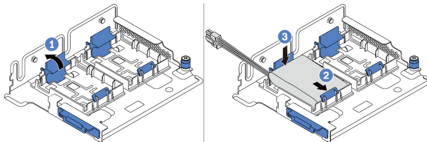
图 155. 安装超级电容器模块
