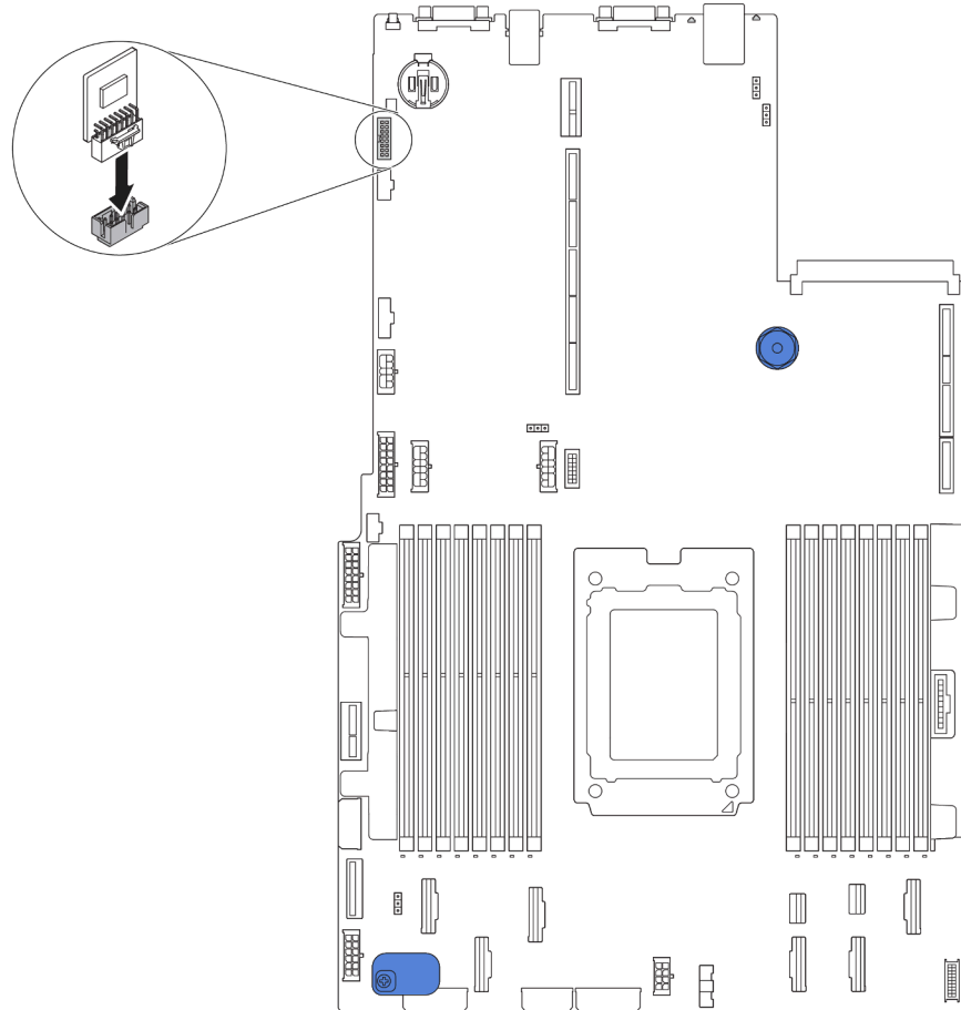
图 128. 安装 TPM 适配器
