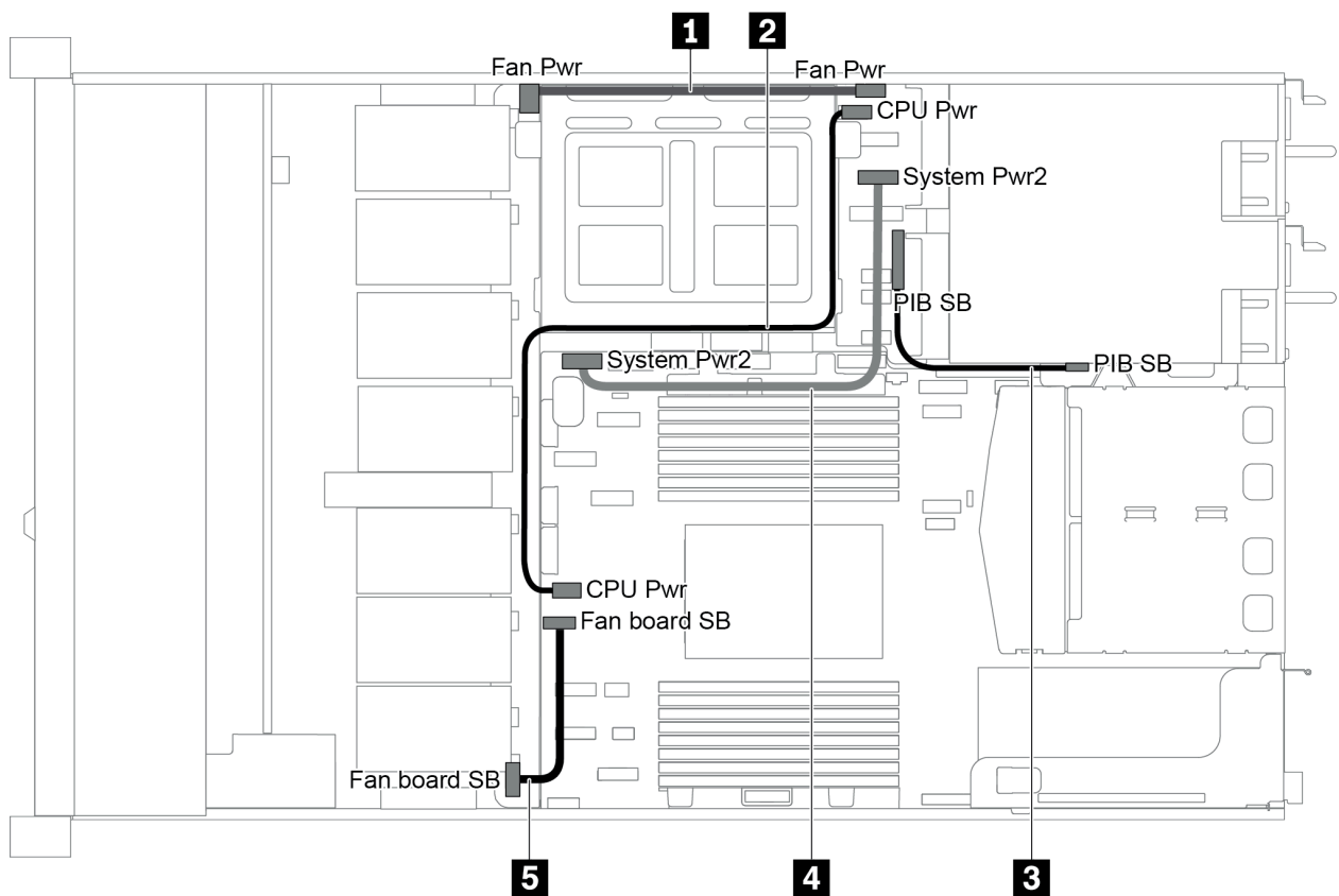
图 20. 2.5 寸机箱 - 1
