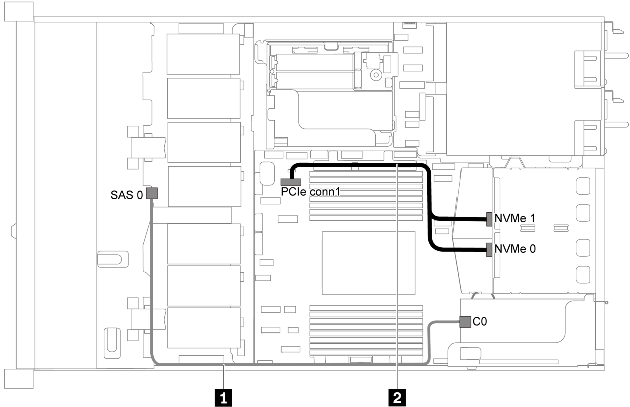
图 29. 配备四个 3.5 英寸 SAS/SATA 硬盘、背面 NVMe 硬盘组合件和一个 8i RAID/HBA 的服务器型号的线缆布放
