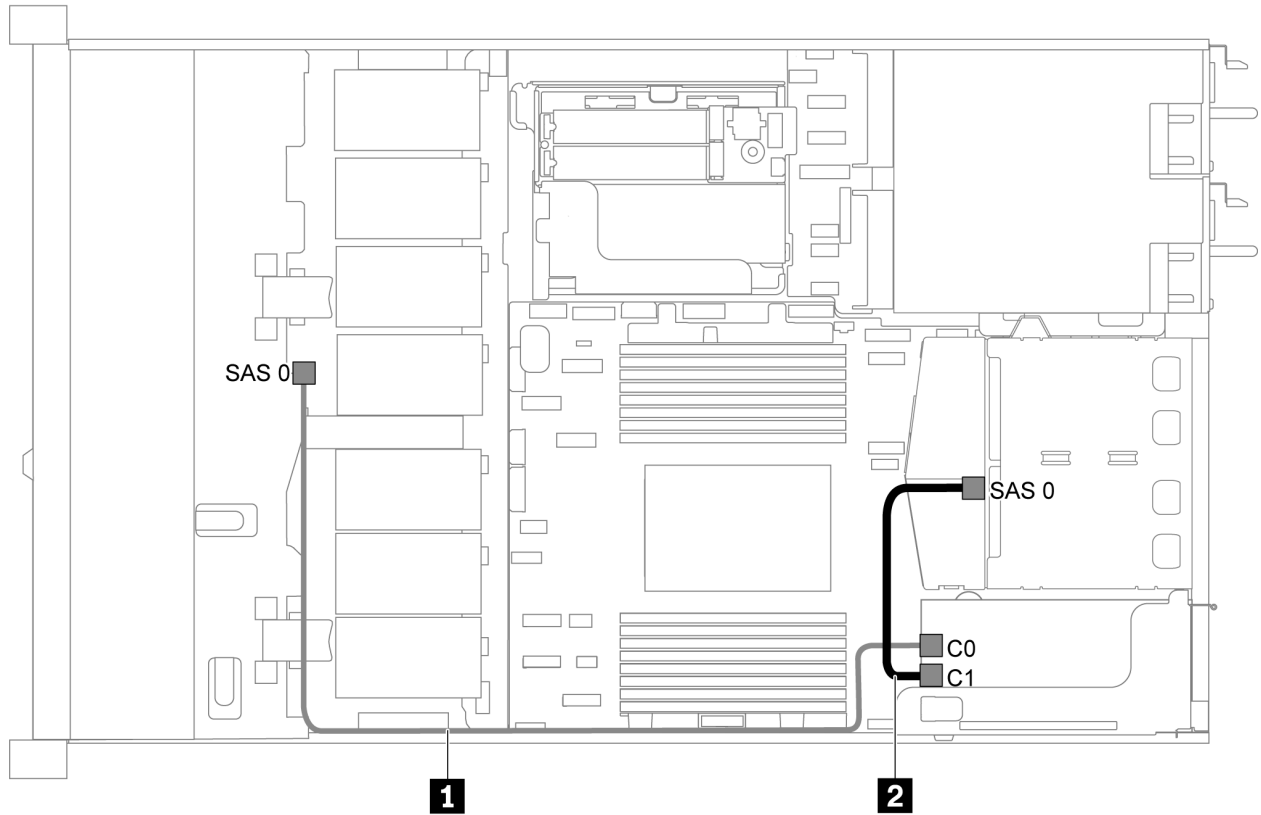
图 27. 配备四个 3.5 英寸 SAS/SATA 硬盘、背面 SAS/SATA 硬盘组合件和一个 8i RAID/HBA 适配器的服务器型号的线缆布放
