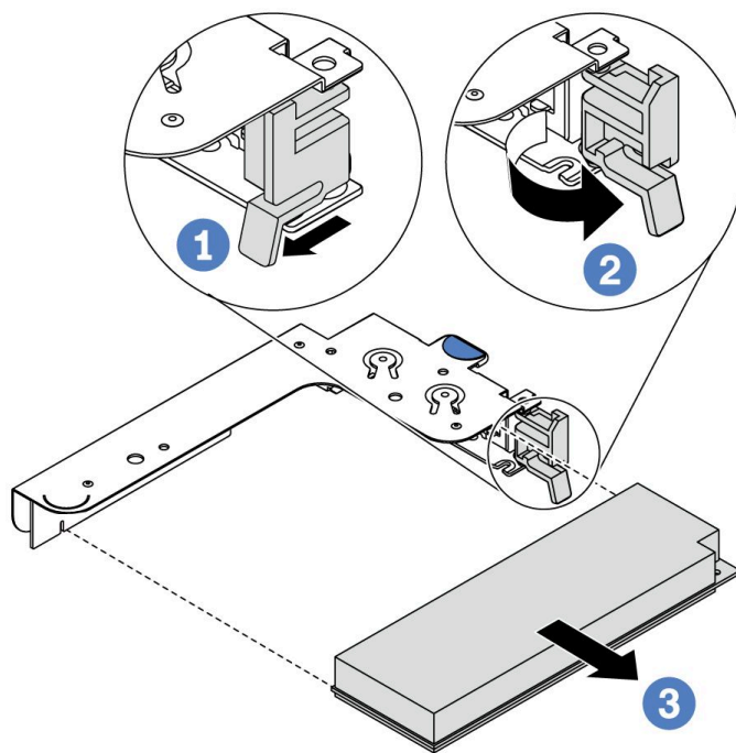
图 107. 卸下内部转接卡组合件 (LP)
