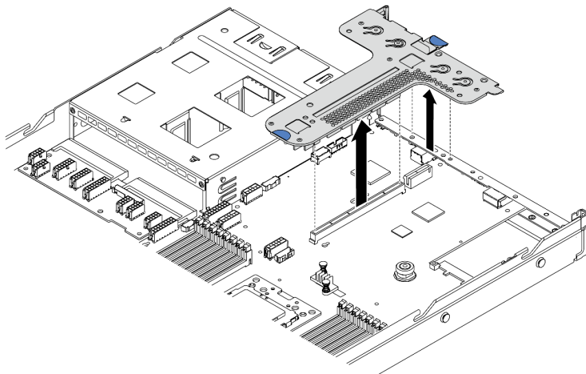
图 100. 卸下转接卡组合件
