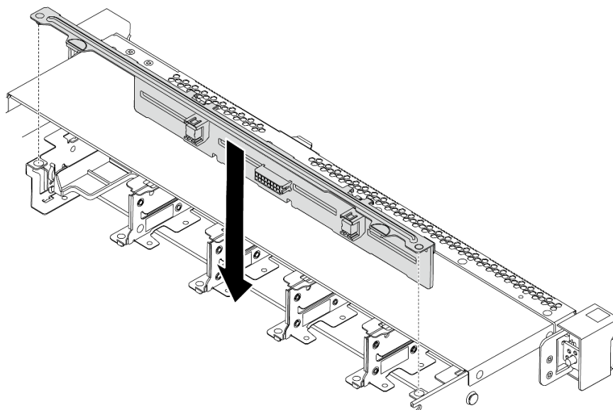
图 116. 安装 8 x 2.5 英寸热插拔硬盘背板
