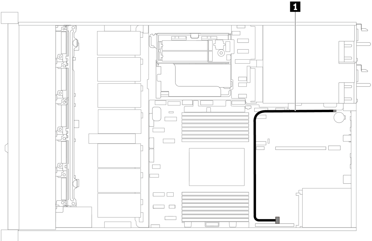
图 65. 配备入侵感应开关的服务器型号的线缆布放
