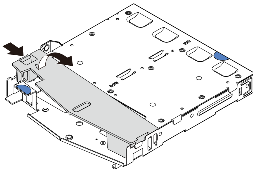
图 130. 卸下导风罩
