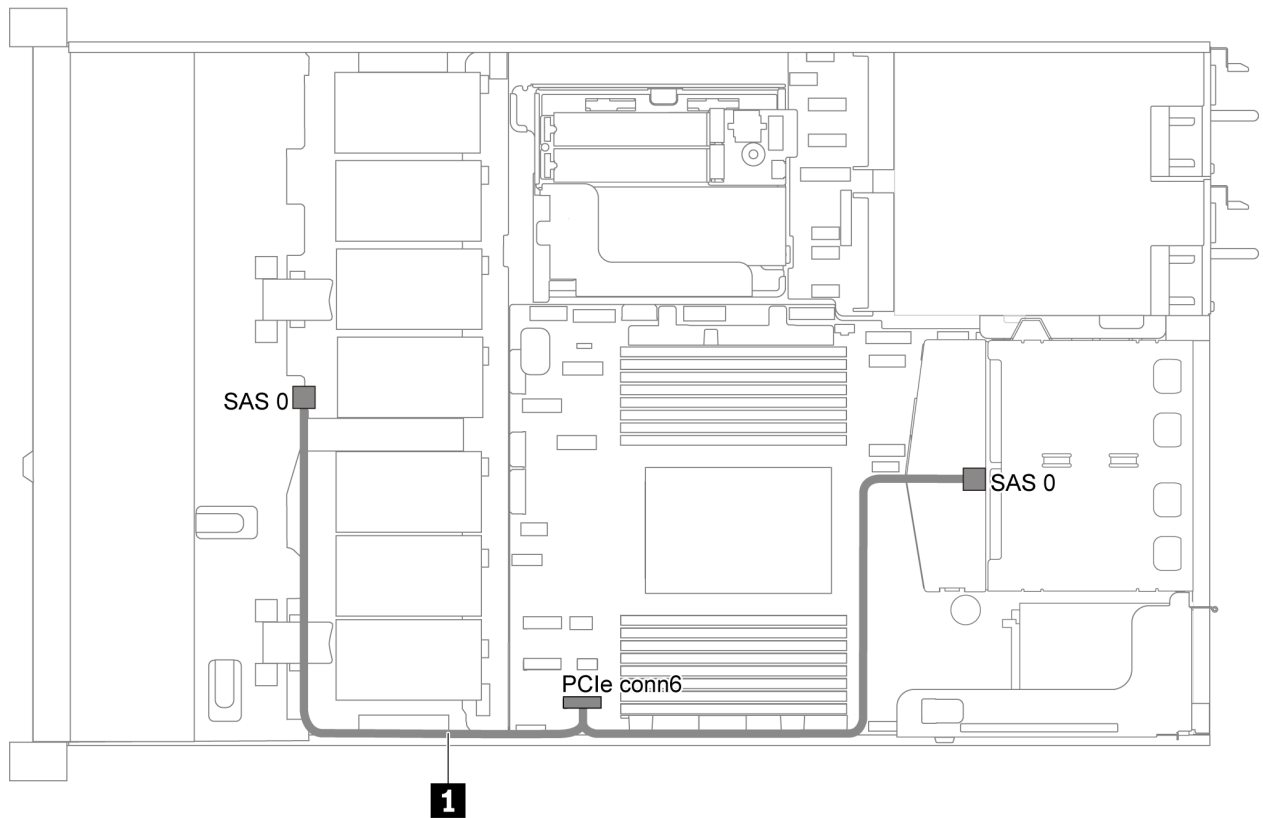
图 26. 配备四个 3.5 英寸 SATA 硬盘和背面 SAS/SATA 硬盘组合件的服务器型号的线缆布放
