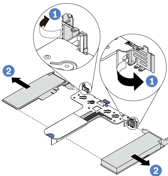
图 106. 卸下转接卡 2 组合件 (LP+LP)
