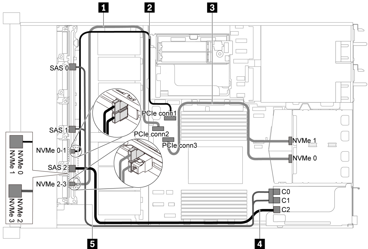
图 46. 配备六个 2.5 英寸 SAS/SATA 硬盘、四个 2.5 英寸 RAID/SATA/NVMe 硬盘、背面 NVMe 硬盘组合件和一个 16i RAID/HBA 适配器的服务器型号的线缆布放
