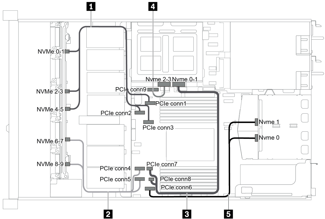
图 55. 配备十个 2.5 英寸 NVMe 硬盘、背面 NVMe 硬盘组合件和中间 NVMe 硬盘组合件的服务器型号的线缆布放
