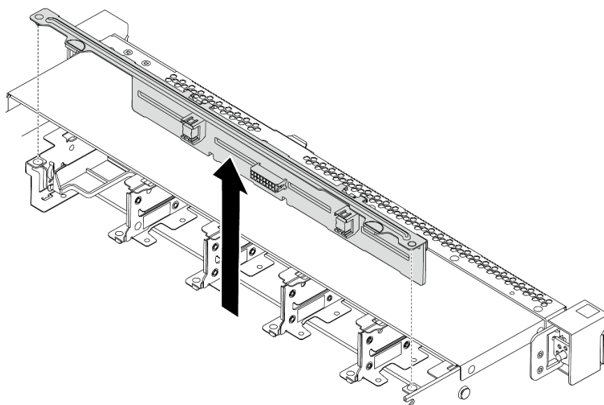
图 115. 卸下 8 x 2.5 英寸热插拔硬盘背板
