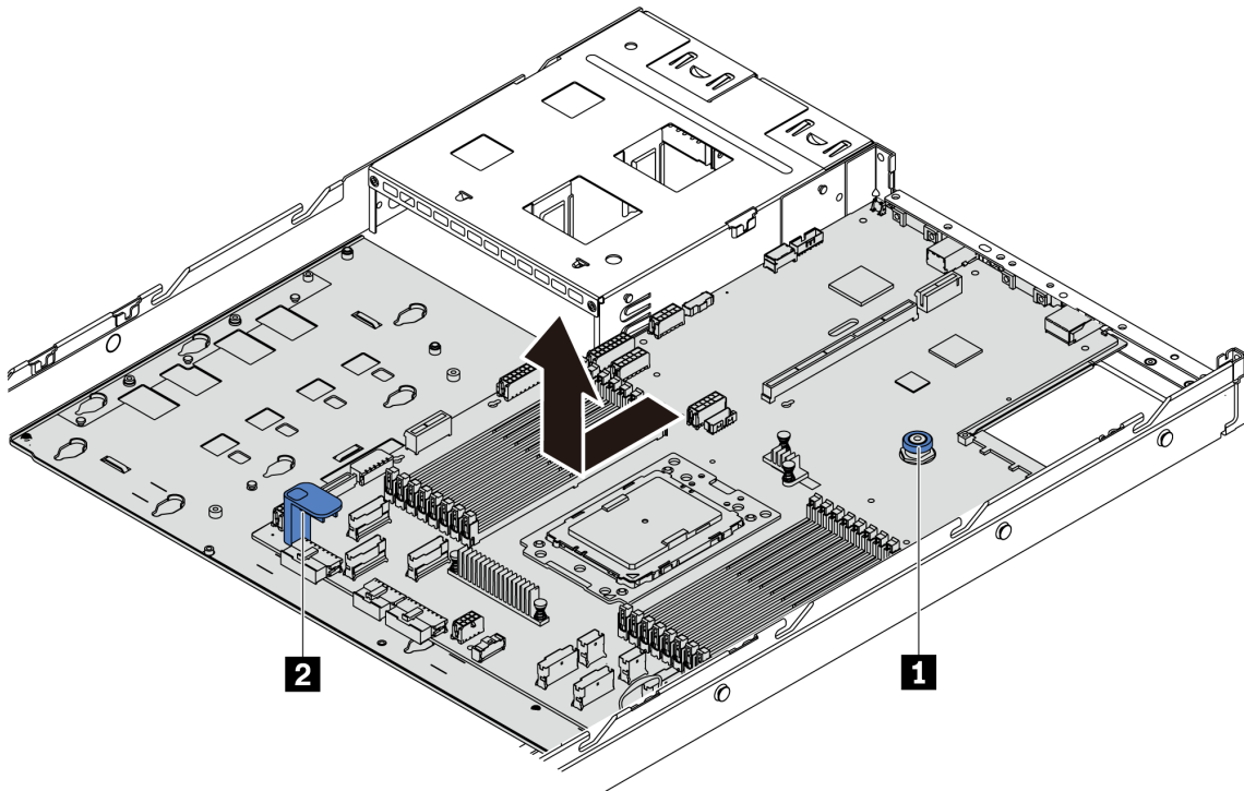
图 181. 卸下主板
