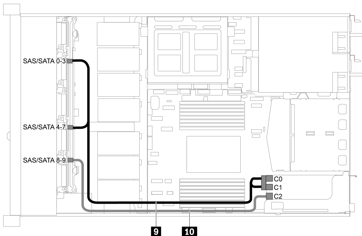
图 57. 配备十个 2.5 英寸 SAS/SATA/NVMe 硬盘、背面 SAS/SATA 硬盘组合件、中间 NVMe 硬盘组合件和一个 16i RAID/HBA 适配器的服务器型号的线缆布放 - 2
