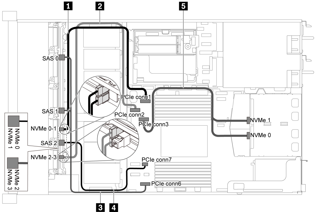
图 45. 配备六个 2.5 英寸 SATA 硬盘、四个 2.5 英寸 NVMe 硬盘和背面 NVMe 硬盘组合件的服务器型号的线缆布放
