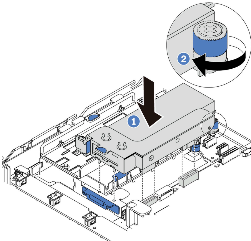
图 96. 安装内部转接卡组合件
