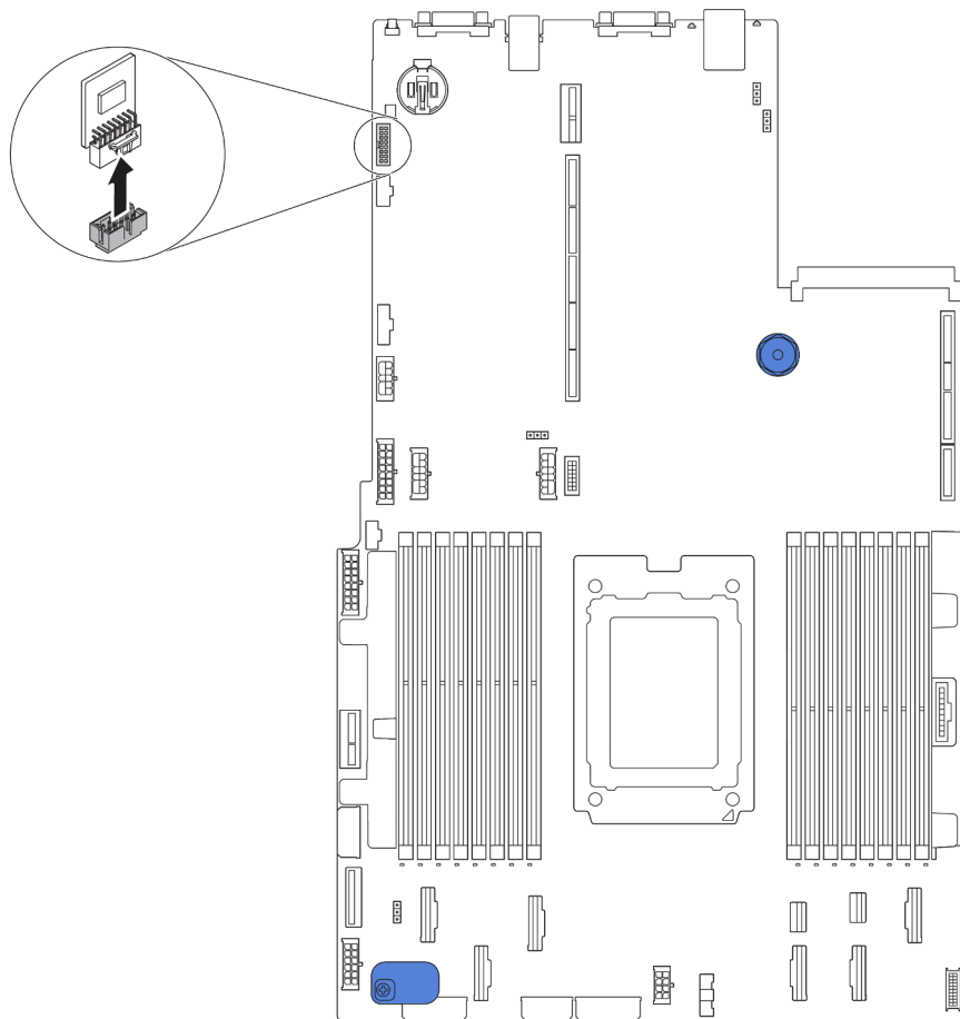
图 127. 卸下 TPM 适配器
