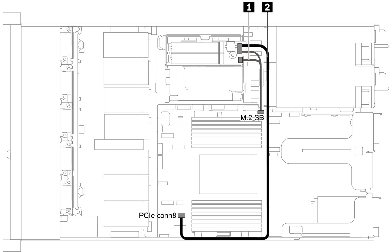
图 60. 配备 M.2 模块的服务器型号的线缆布放
