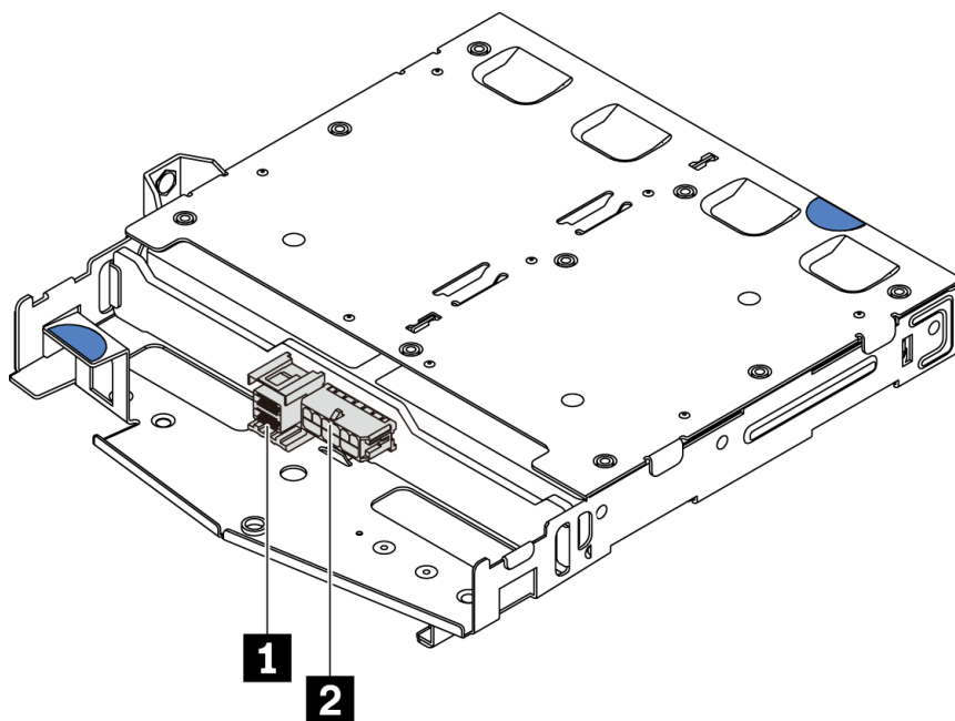
图 123. SAS/SATA 背面背板接口
