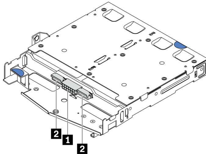
图 132. NVMe 背面背板接口
