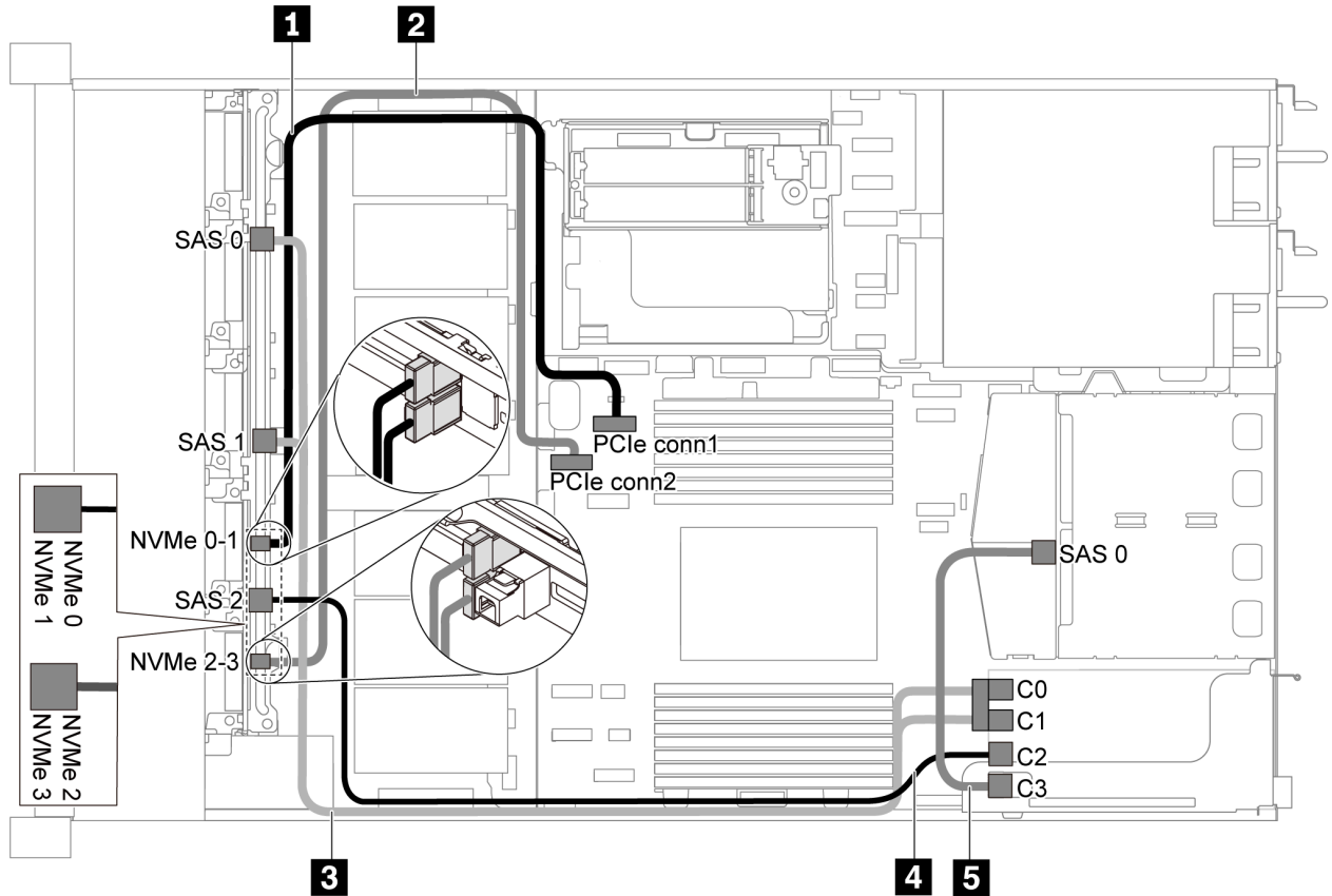
图 44. 配备六个 2.5 英寸 SAS/SATA 硬盘、四个 2.5 英寸 NVMe 硬盘、背面 SAS/SATA 硬盘组合件和一个 16i RAID/HBA 适配器的服务器型号的线缆布放
