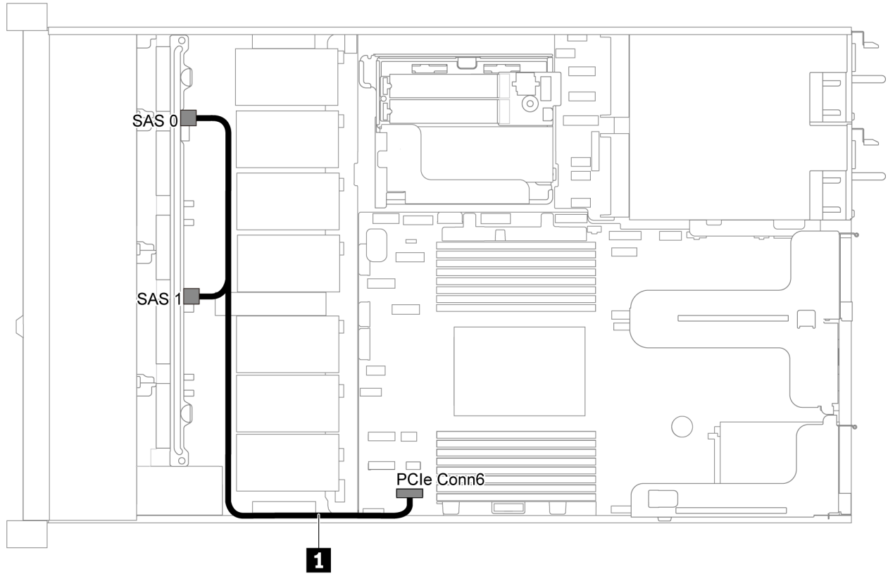
图 33. 配备八个 2.5 英寸 SATA 硬盘的服务器型号的线缆布放
