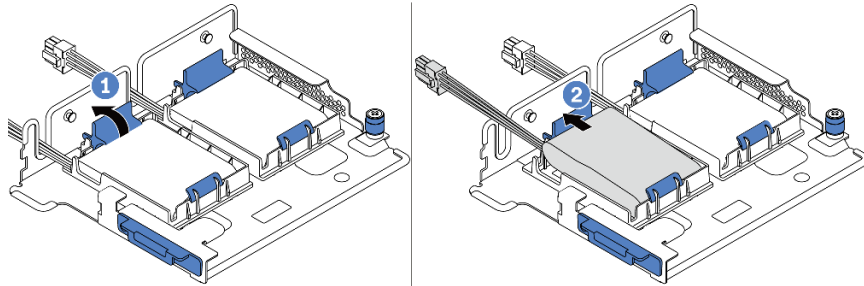
图 154. 卸下超级电容器模块
