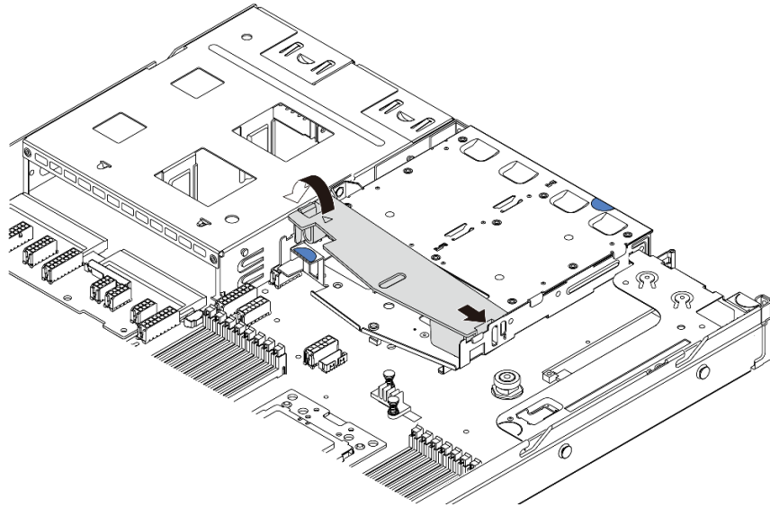
图 124. 安装导风罩
