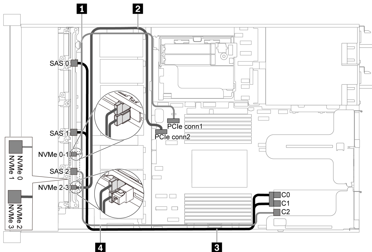
图 42. 配备六个 2.5 英寸 SAS/SATA 硬盘、四个 2.5 英寸 NVMe 硬盘和一个 16i RAID/HBA 适配器的服务器型号的线缆布放
