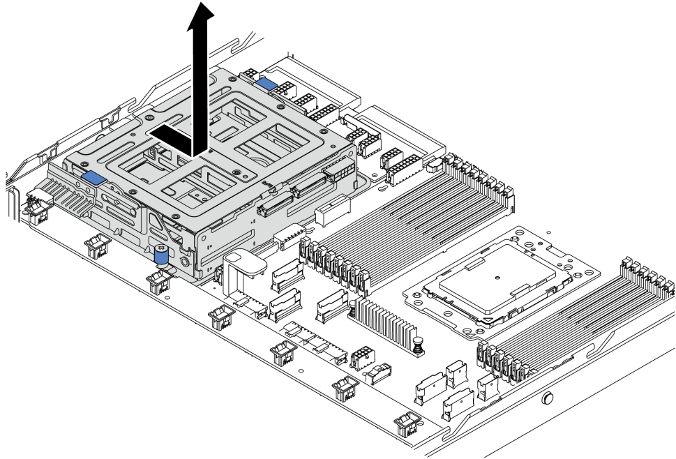
图 139. 卸下中间硬盘仓 - 2
