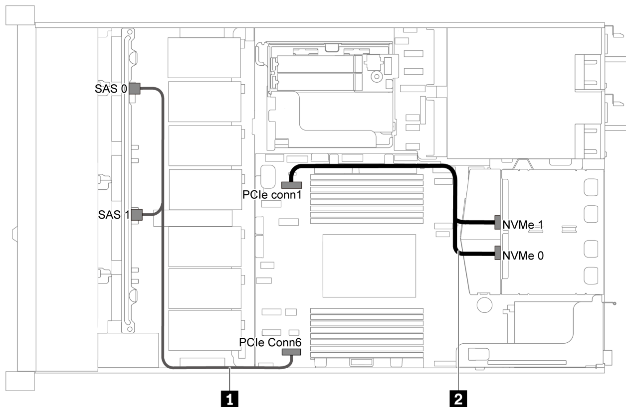
图 38. 配备八个 2.5 英寸 SATA 硬盘和背面 NVMe 硬盘组合件的服务器型号的线缆布放
