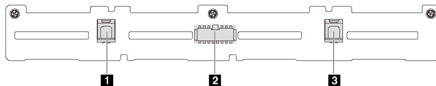
图 32. 用于八个 2.5 英寸 SAS/SATA 硬盘的背板上的接口
