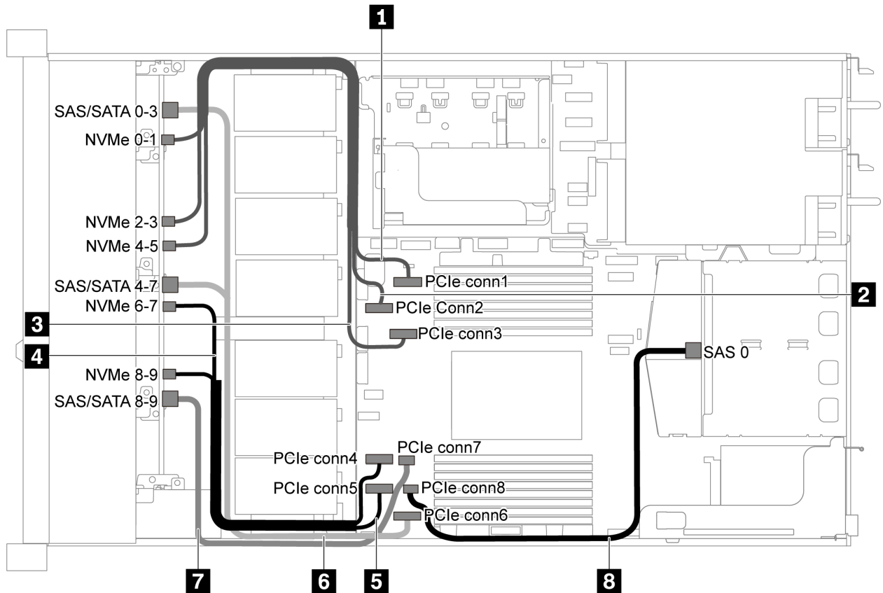
图 50. 配备十个 2.5 英寸 SATA/NVMe 硬盘和背面 SAS/SATA 硬盘组合件的服务器型号的线缆布放
