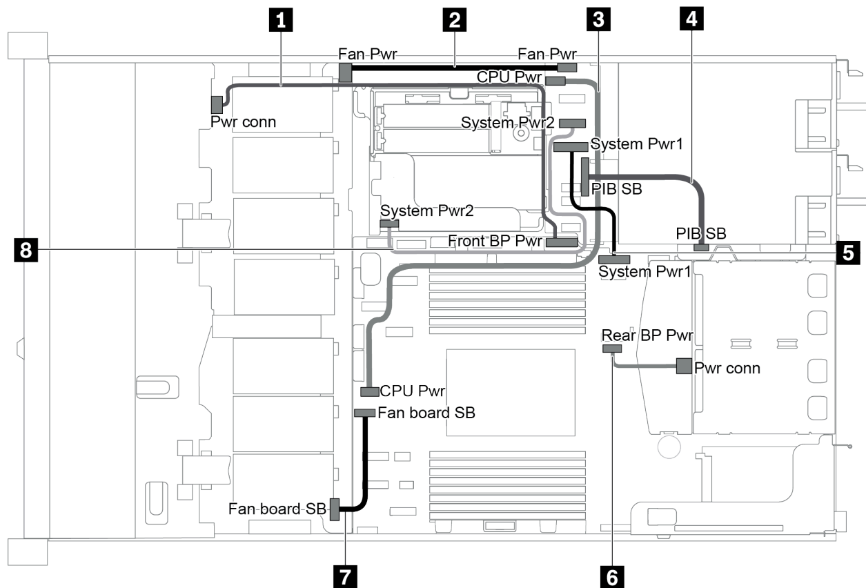
图 22. 3.5 寸机箱
