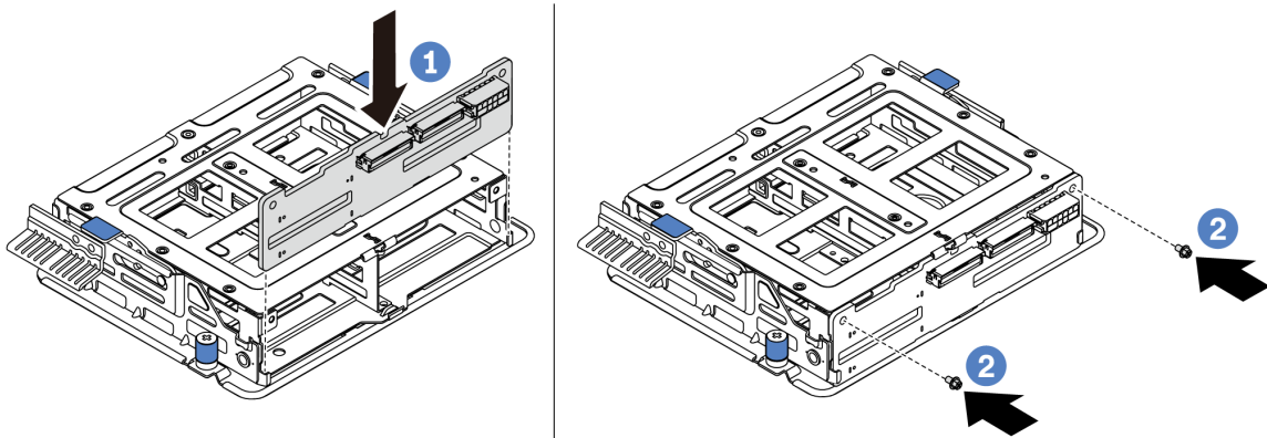
图 141. 安装内部背板
