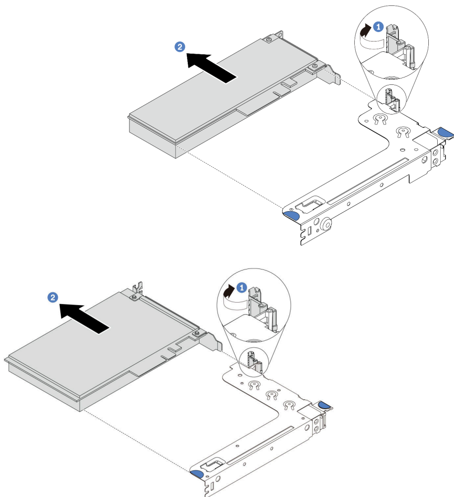
图 105. 卸下转接卡 1 组合件 (LP/FHFL)
