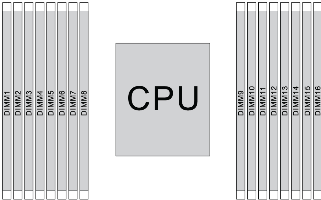
图 67. DIMM 位置
