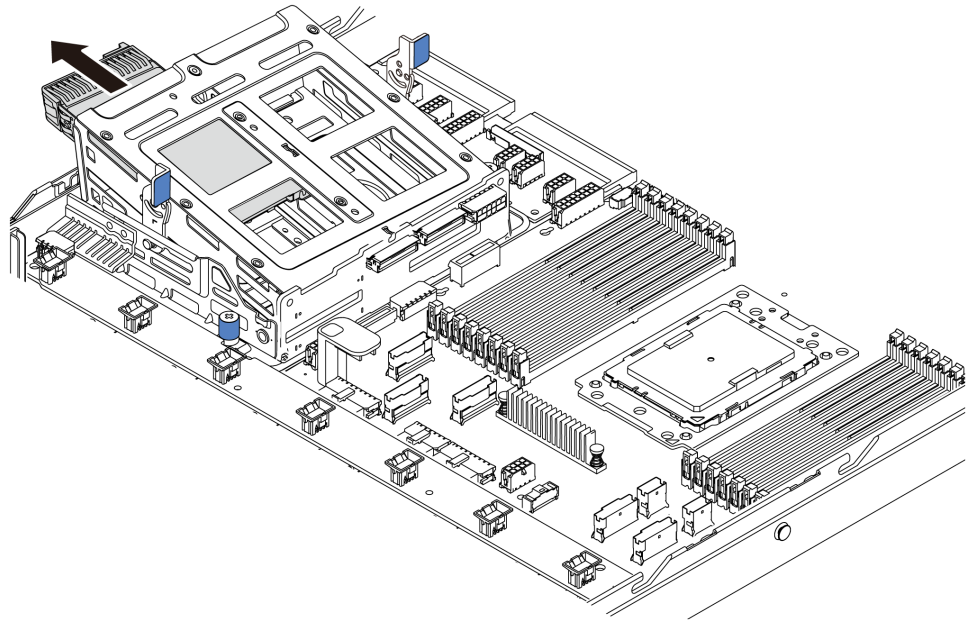
图 137. 卸下内部硬盘 - 2
