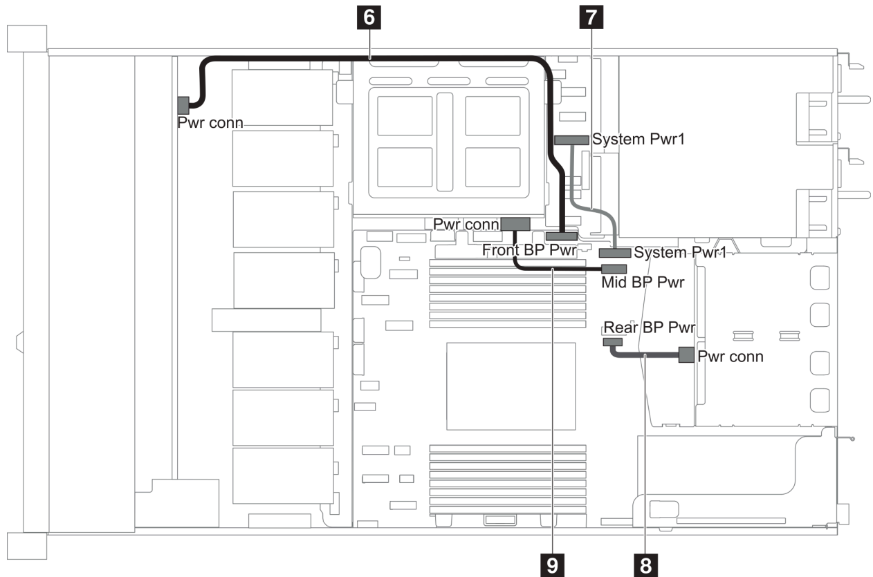
图 21. 2.5 寸机箱 - 2
