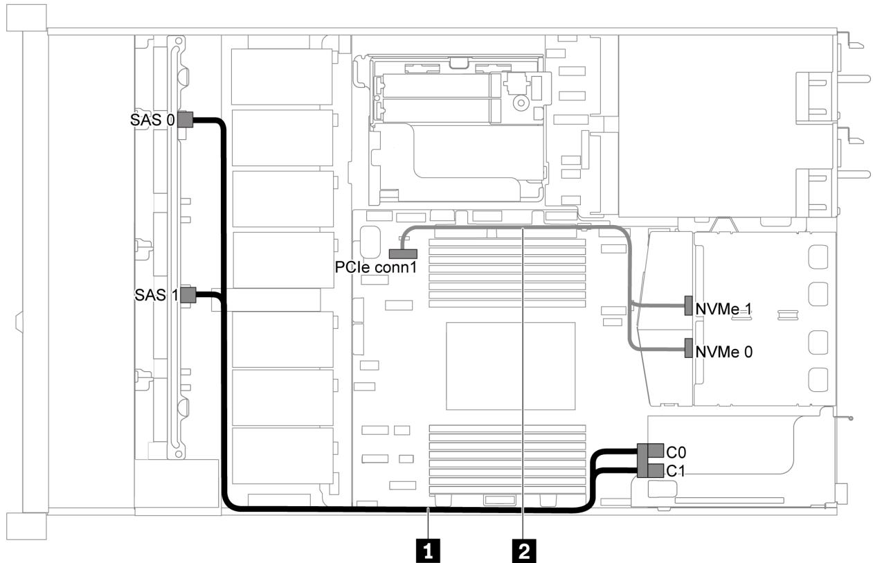
图 39. 配备八个 2.5 英寸 SAS/SATA 硬盘、背面 NVMe 硬盘组合件和一个 8i RAID/HBA 的服务器型号的线缆布放
