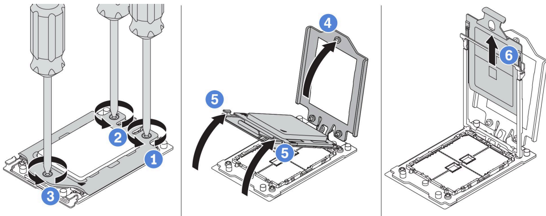
图 173. 卸下处理器
