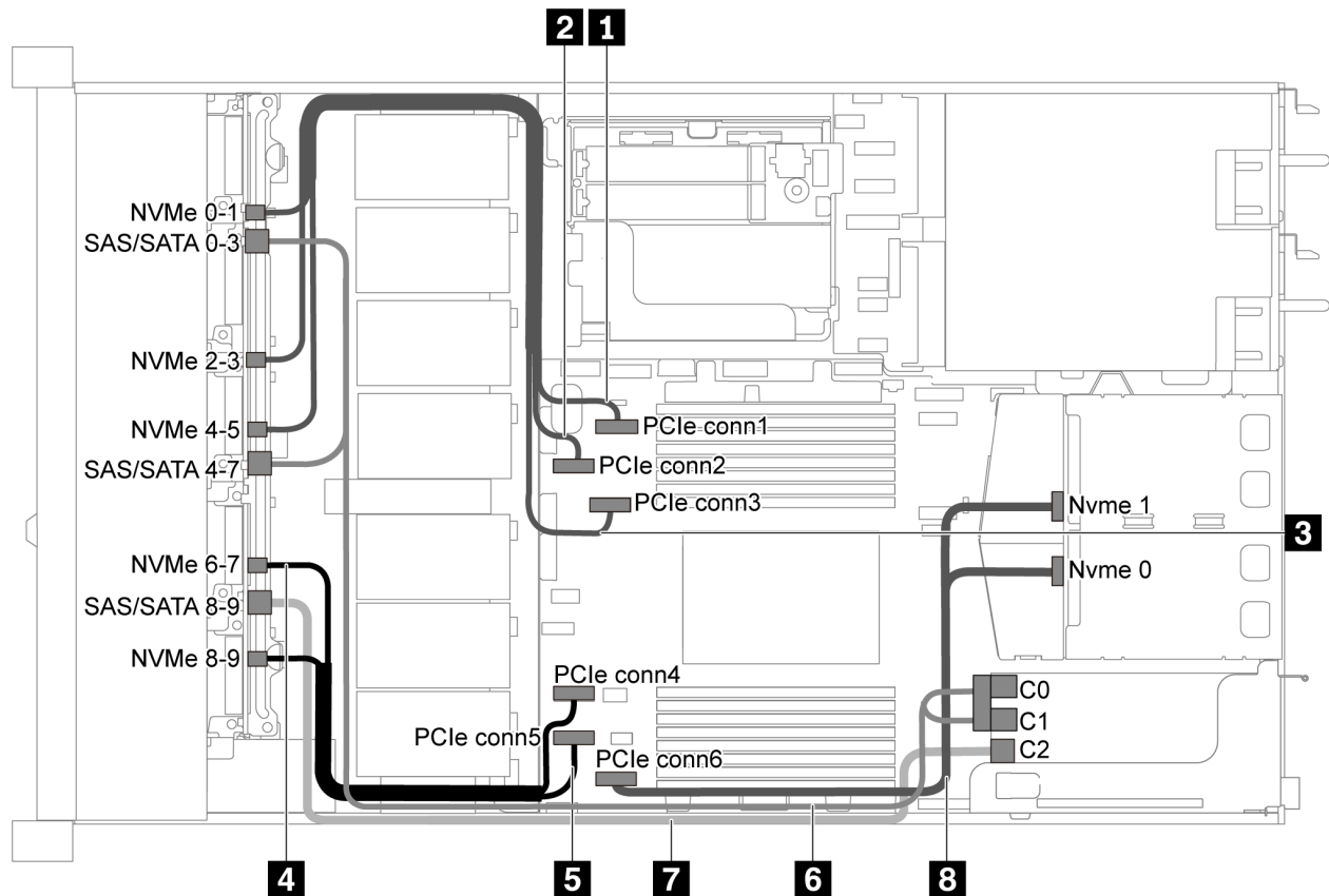
图 52. 配备十个 2.5 英寸 SAS/SATA/NVMe 硬盘、背面 NVMe 硬盘组合件和一个 16i RAID/HBA 适配器的服务器型号的线缆布放
