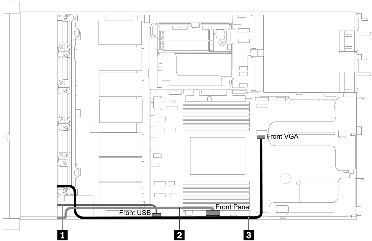
图 64. 配备八个/十个 2.5 英寸硬盘插槽的服务器型号的 VGA/USB/前面板接口线缆布放
