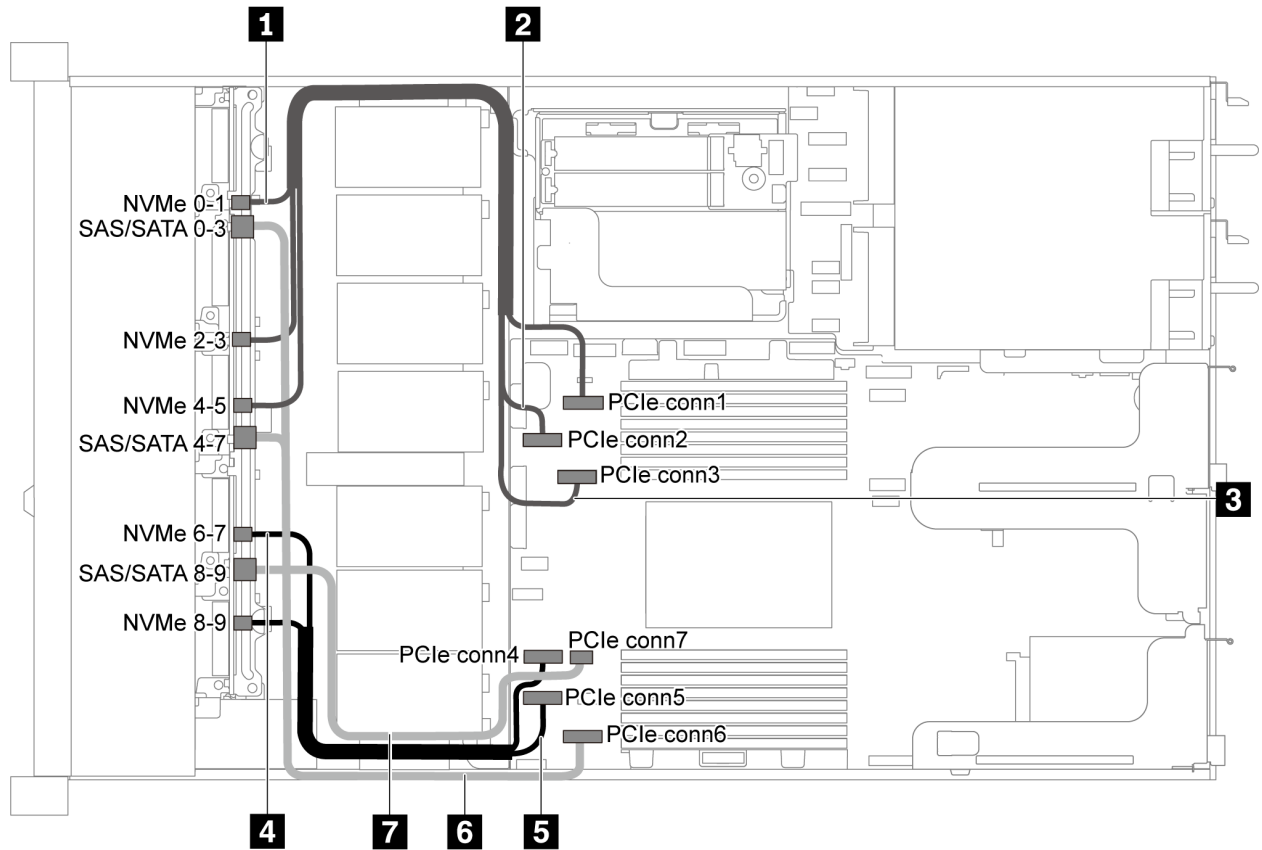
图 48. 配备十个 2.5 英寸 SATA/NVMe 硬盘的服务器型号的线缆布放
