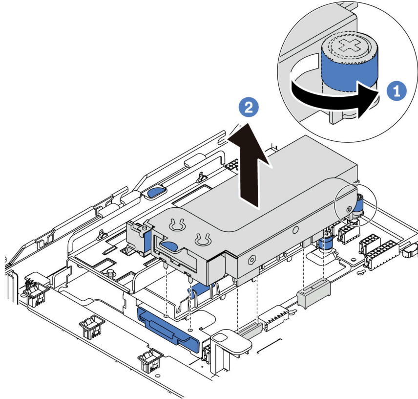
图 95. 卸下内部转接卡组合件
