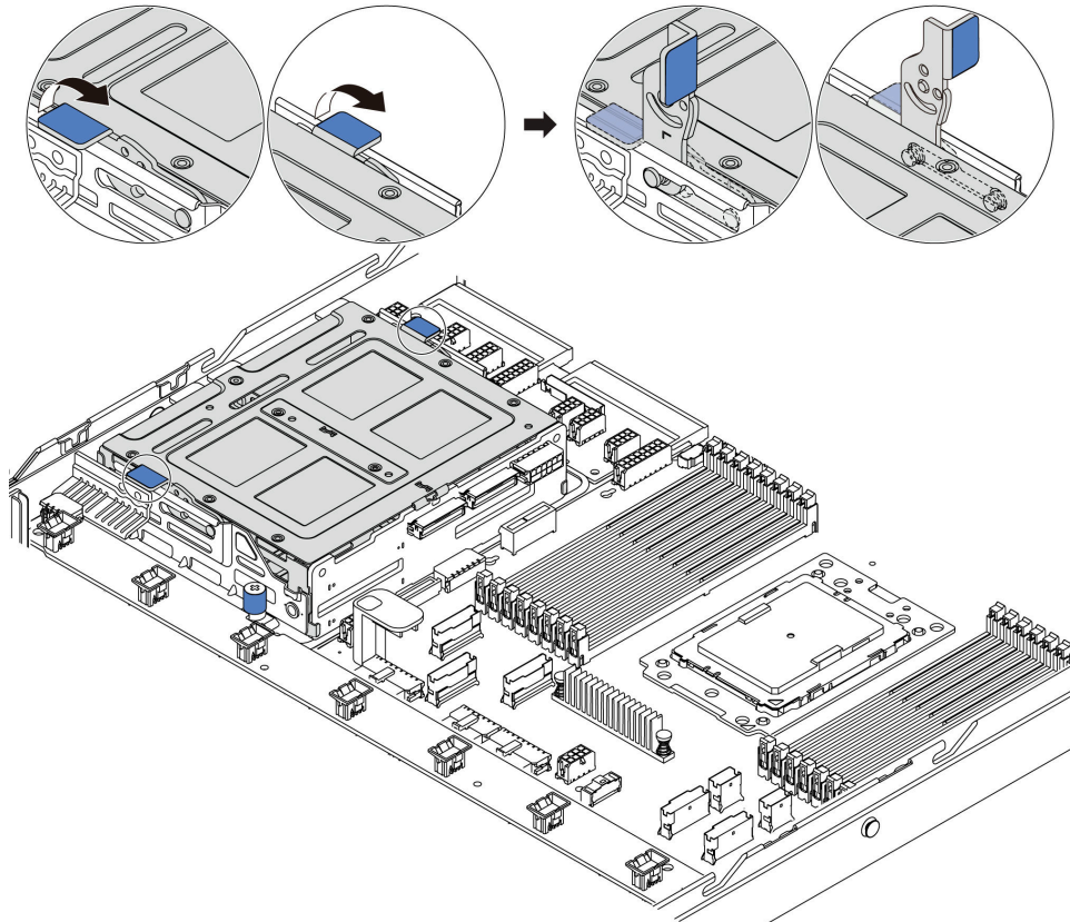
图 136. 卸下内部硬盘 - 1
