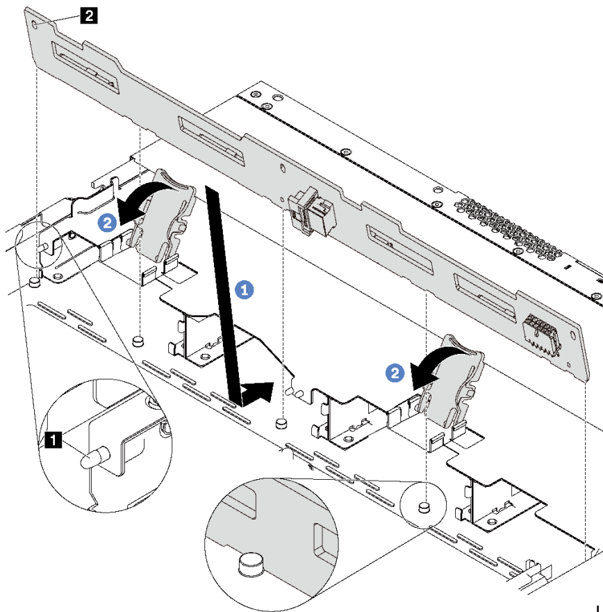
图 114. 安装 4 x 3.5 英寸热插拔硬盘背板
