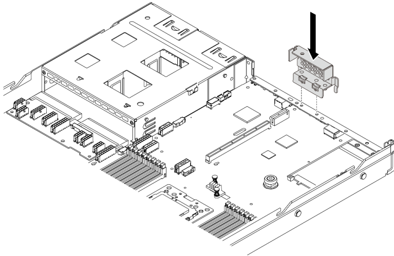
图 104. 安装背面壁挂支架
