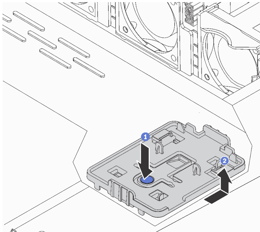
图 158. 卸下托盘
