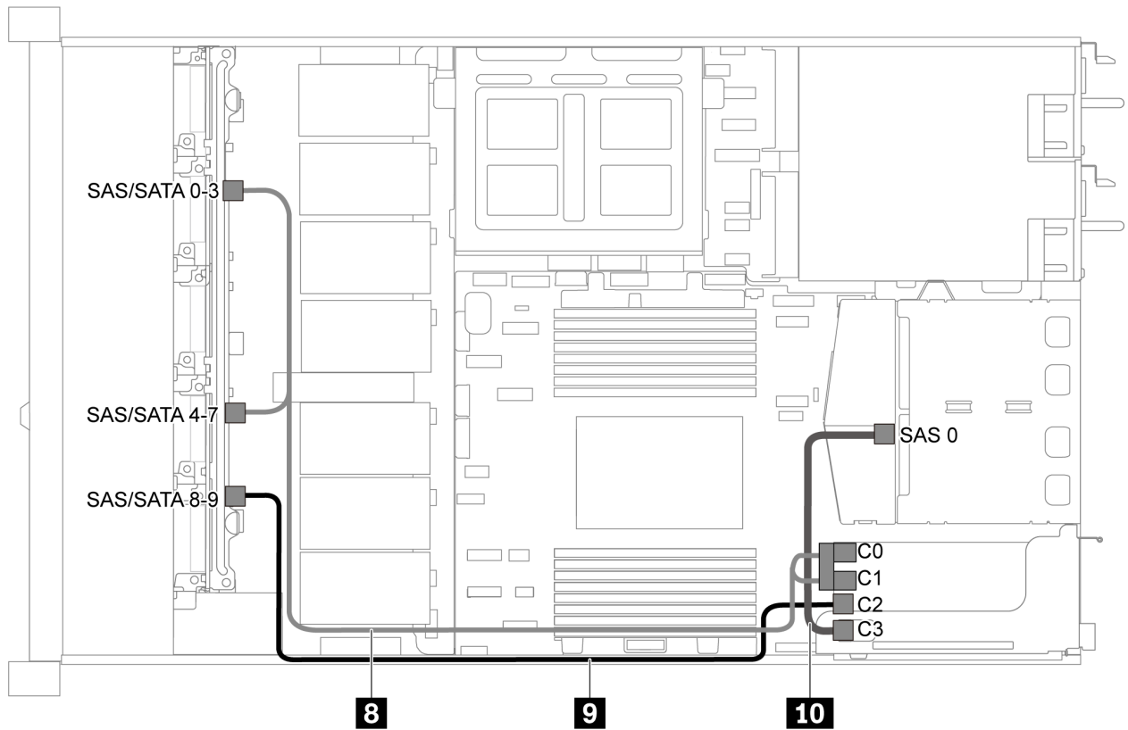
图 54. 配备十个 2.5 英寸 SAS/SATA/NVMe 硬盘、背面 SAS/SATA 硬盘组合件、中间 NVMe 硬盘组合件和一个 16i RAID/HBA 适配器的服务器型号的线缆布放 - 2
