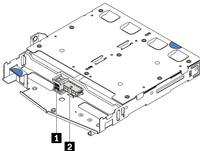
图 133. SAS/SATA 背面背板接口
