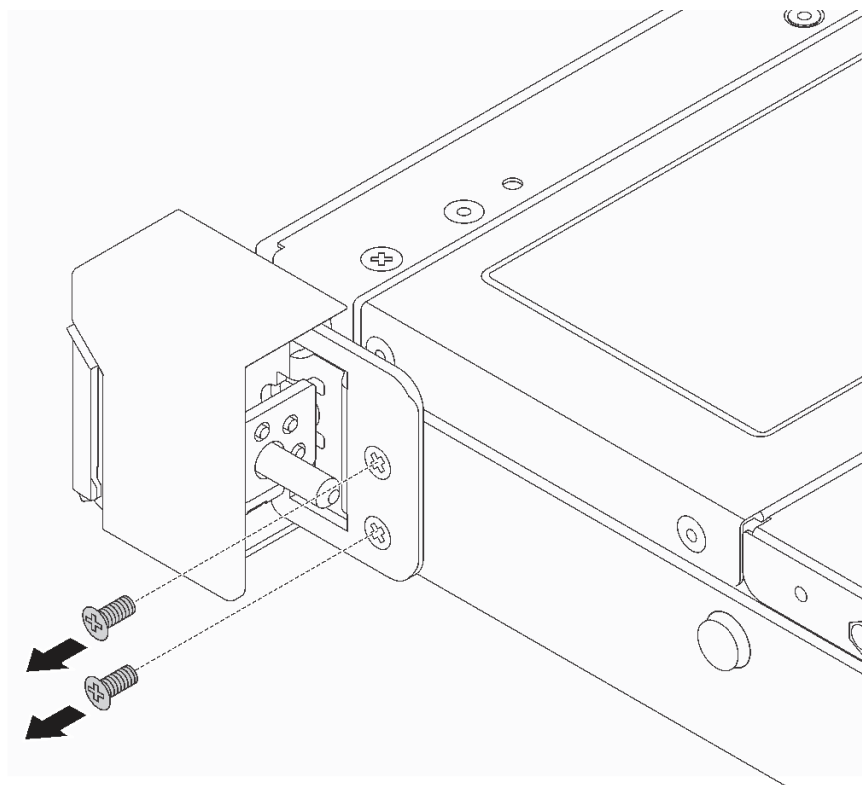
图 73. 卸下机架滑锁螺钉
