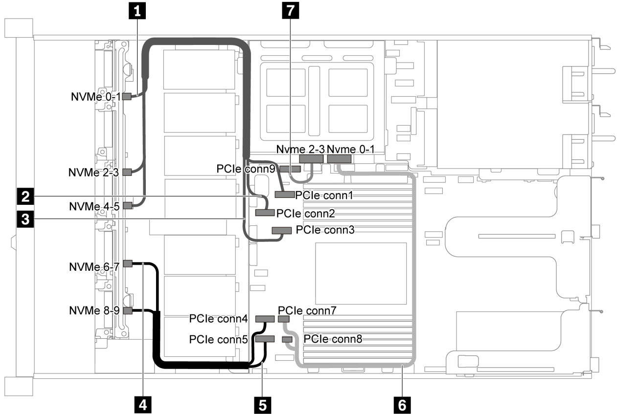
图 58. 配备十个 2.5 英寸 SAS/SATA/NVMe 硬盘、中间 NVMe 硬盘组合件和一个 16i RAID/HBA 适配器的服务器型号的线缆布放 - 1
