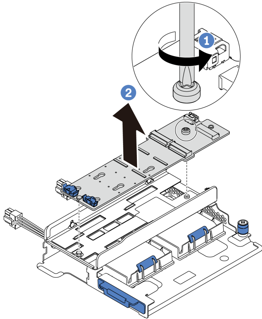
图 147. 卸下 M.2 适配器
