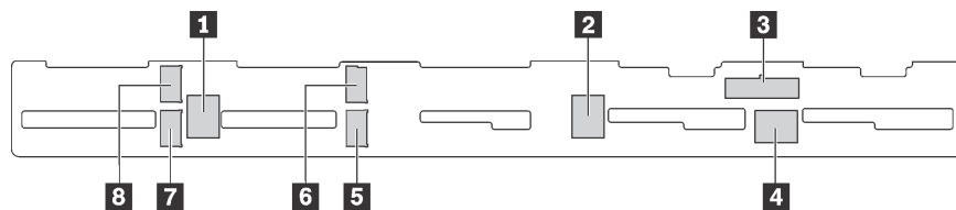
图 40. 用于六个 2.5 英寸 SAS/SATA 硬盘和四个 2.5 英寸 NVMe 硬盘的背板上的接口
