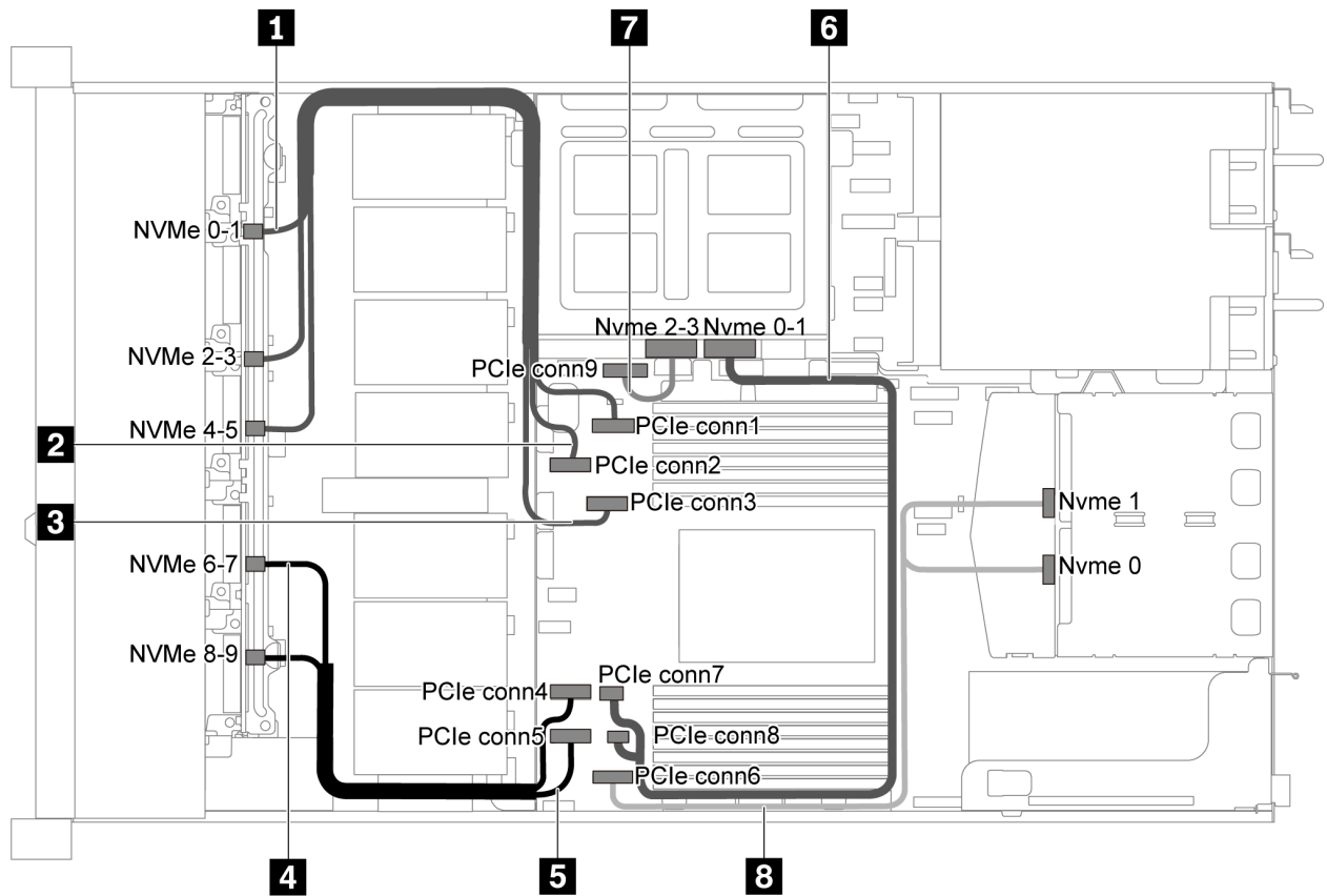
图 56. 配备十个 2.5 英寸 SAS/SATA/NVMe 硬盘、背面 NVMe 硬盘组合件、中间 NVMe 硬盘组合件和一个 16i RAID/HBA 适配器的服务器型号的线缆布放 - 1
