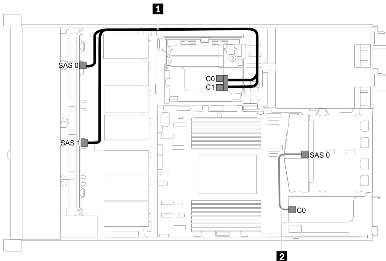
图 36. 配备八个 2.5 英寸 SAS/SATA 硬盘、背面 SAS/SATA 硬盘组合件和两个 8i RAID/HBA 适配器的服务器型号的线缆布放
