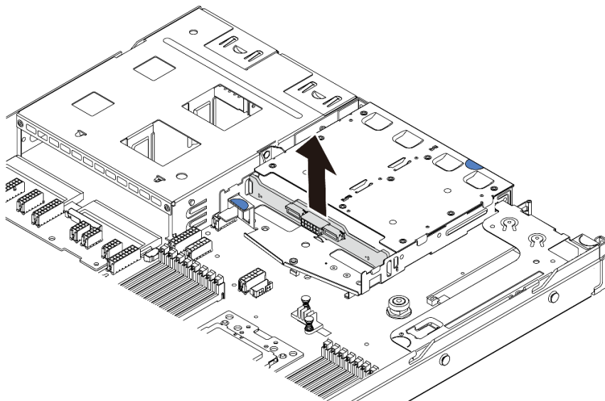
图 120. 卸下背面背板
