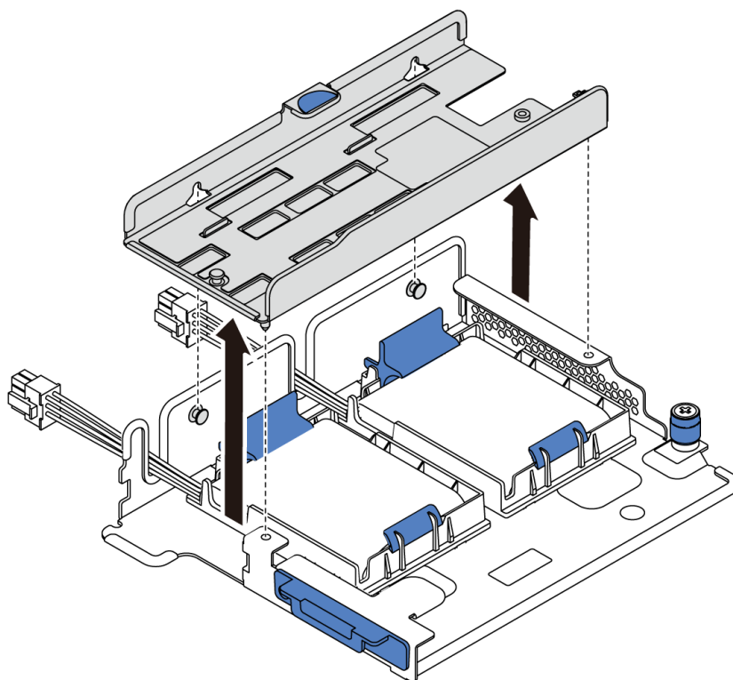
图 148. 卸下 M.2 适配器支架
