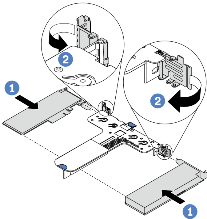
图 109. 安装转接卡 2 组合件 (LP+LP)
