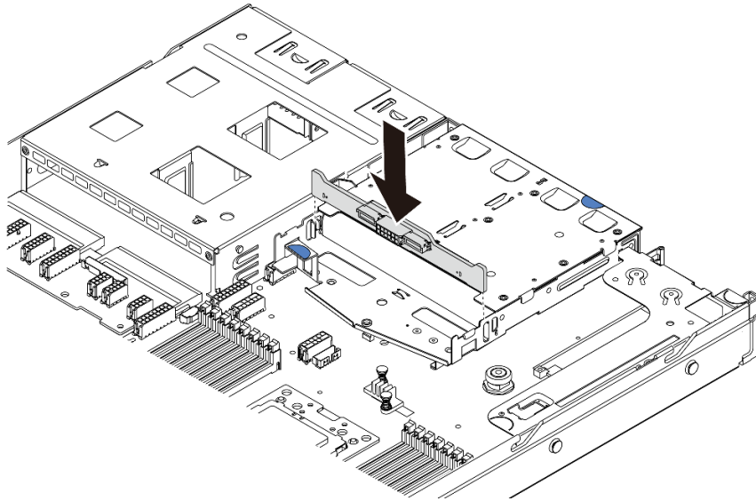
图 131. 安装背面背板
