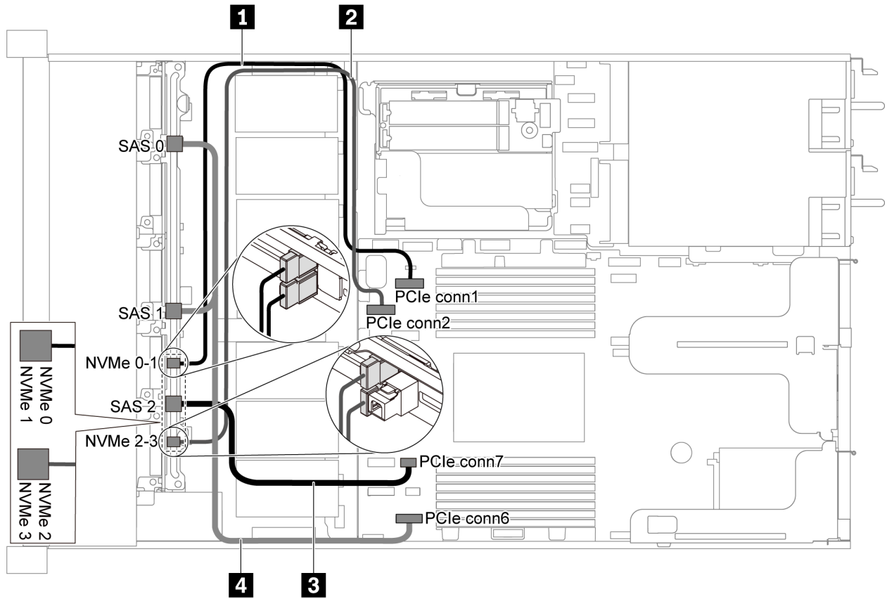
图 41. 配备六个 2.5 英寸 SATA 硬盘和四个 2.5 英寸 NVMe 硬盘的服务器型号的线缆布放
