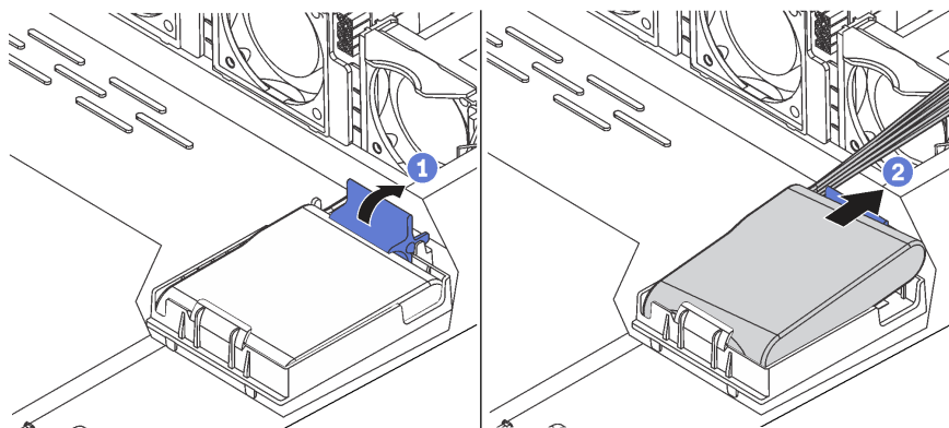
图 156. 卸下机箱上的 RAID 超级电容器模块
