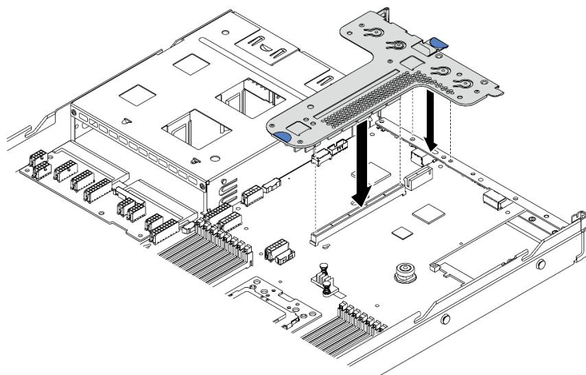
图 103. 安装转接卡组合件
