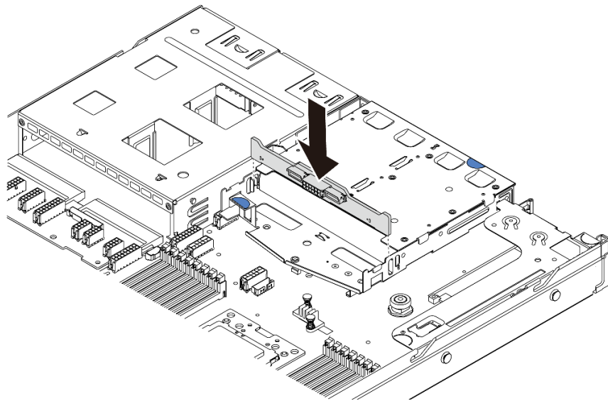
图 121. 安装背面背板
