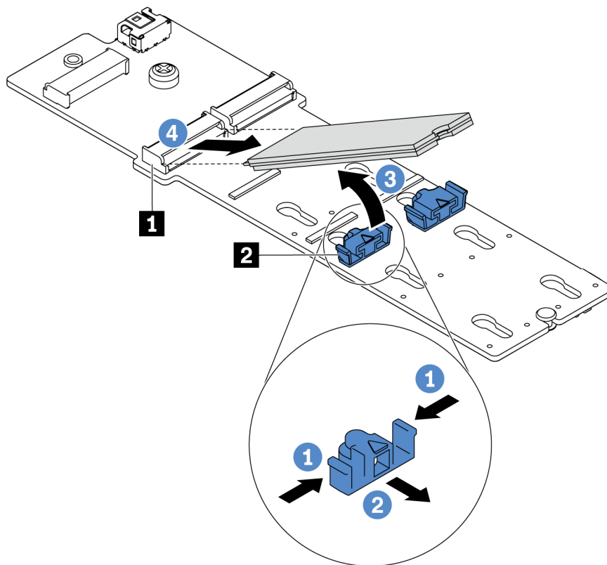
图 146. 卸下 M.2 硬盘
