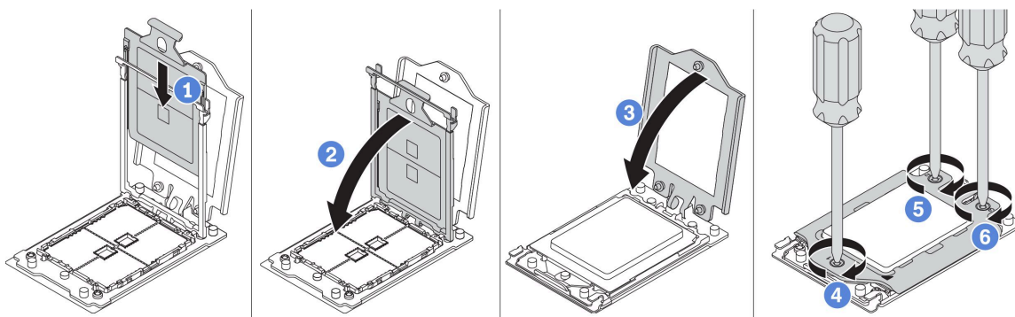
图 174. 安装处理器
