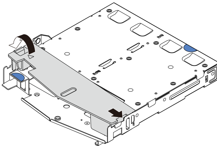
图 134. 安装导风罩
