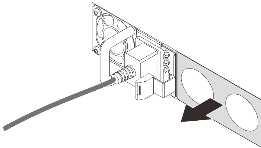
图 170. 卸下热插拔电源模块填充件
