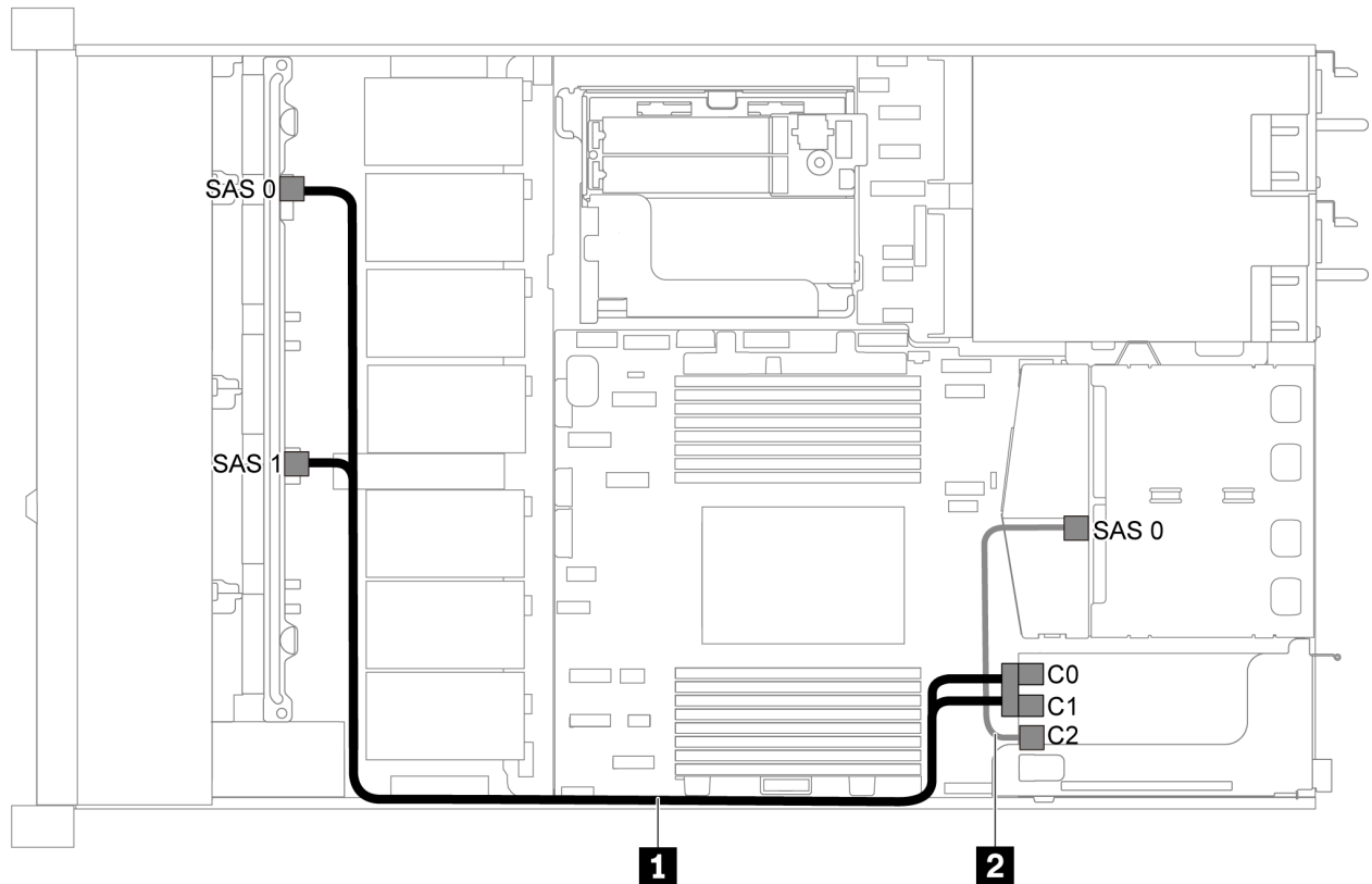
图 37. 配备八个 2.5 英寸 SAS/SATA 硬盘、背面 SAS/SATA 硬盘组合件和一个 16i RAID/HBA 适配器的服务器型号的线缆布放
