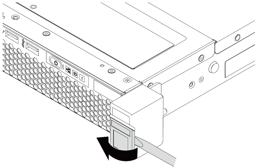
图 72. 卸下标识标签板
