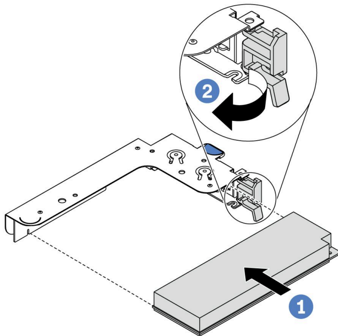
图 110. 安装内部转接卡组合件 (LP)
