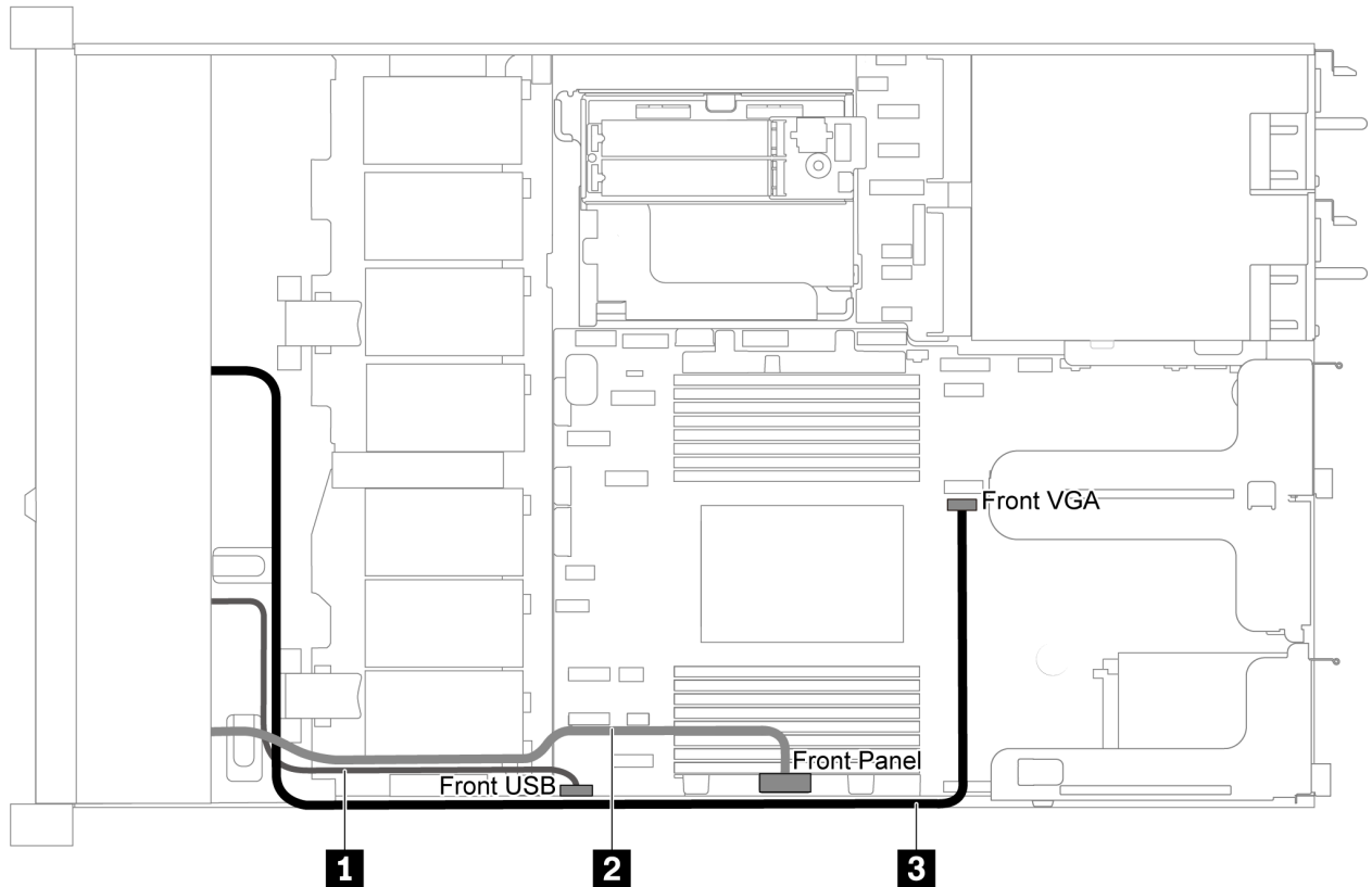
图 63. 配备四个 3.5 英寸硬盘插槽的服务器型号的 VGA/USB/前面板接口线缆布放
