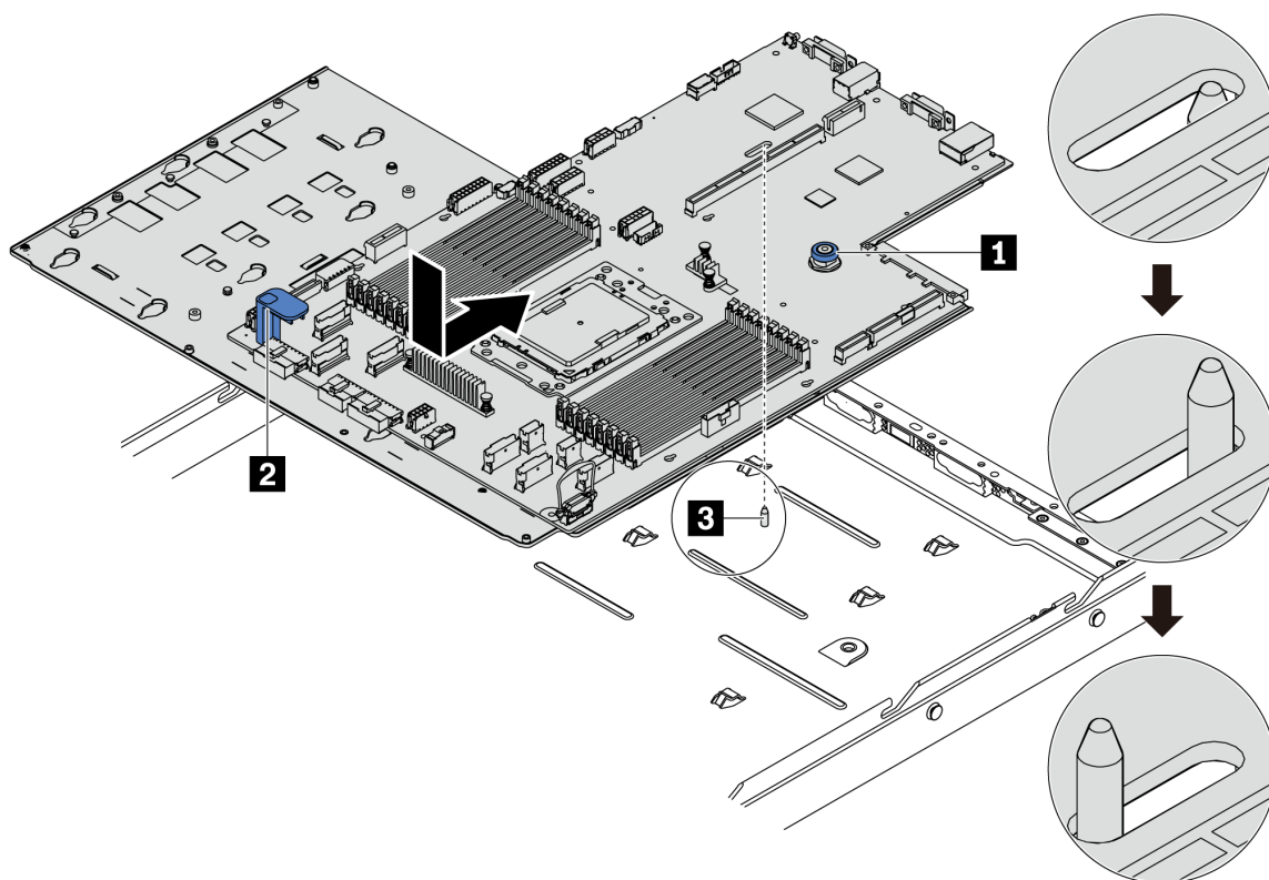
图 182. 安装主板
