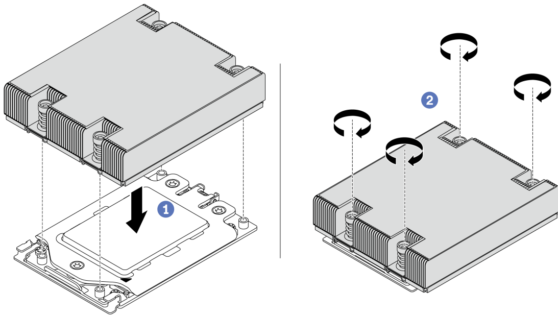
图 176. 安装散热器
