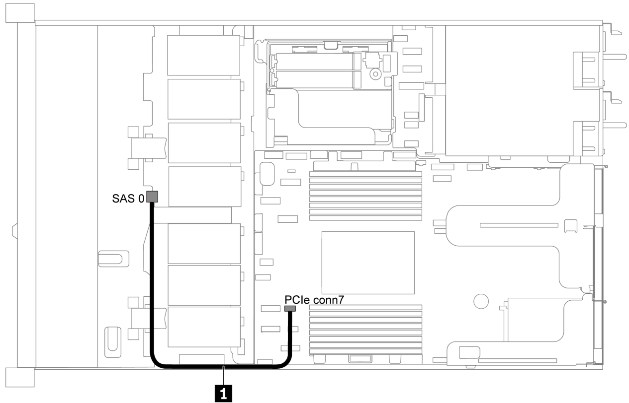
图 24. 配备四个 3.5 英寸 SATA 硬盘的服务器型号的线缆布放
