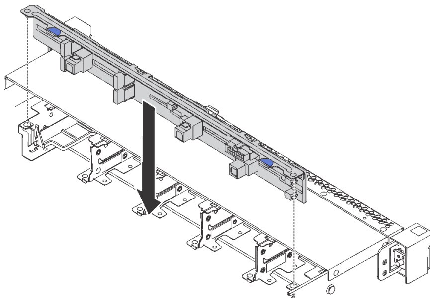
图 118. 安装 10 x 2.5 英寸热插拔硬盘背板
