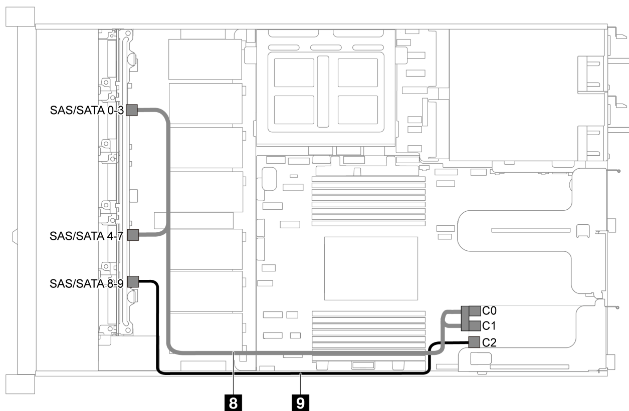
图 59. 配备十个 2.5 英寸 SAS/SATA/NVMe 硬盘、中间 NVMe 硬盘组合件和一个 16i RAID/HBA 适配器的服务器型号的线缆布放 - 2
