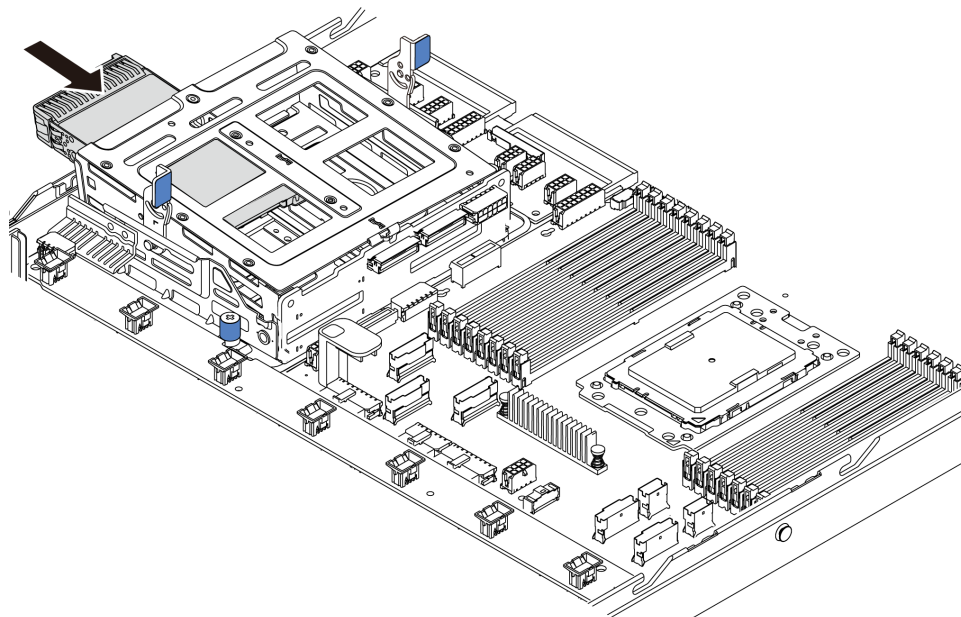
图 144. 安装热插拔硬盘 - 1
