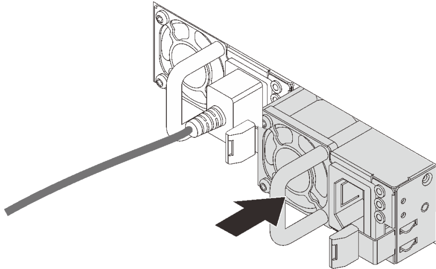
图 171. 安装热插拔电源模块
