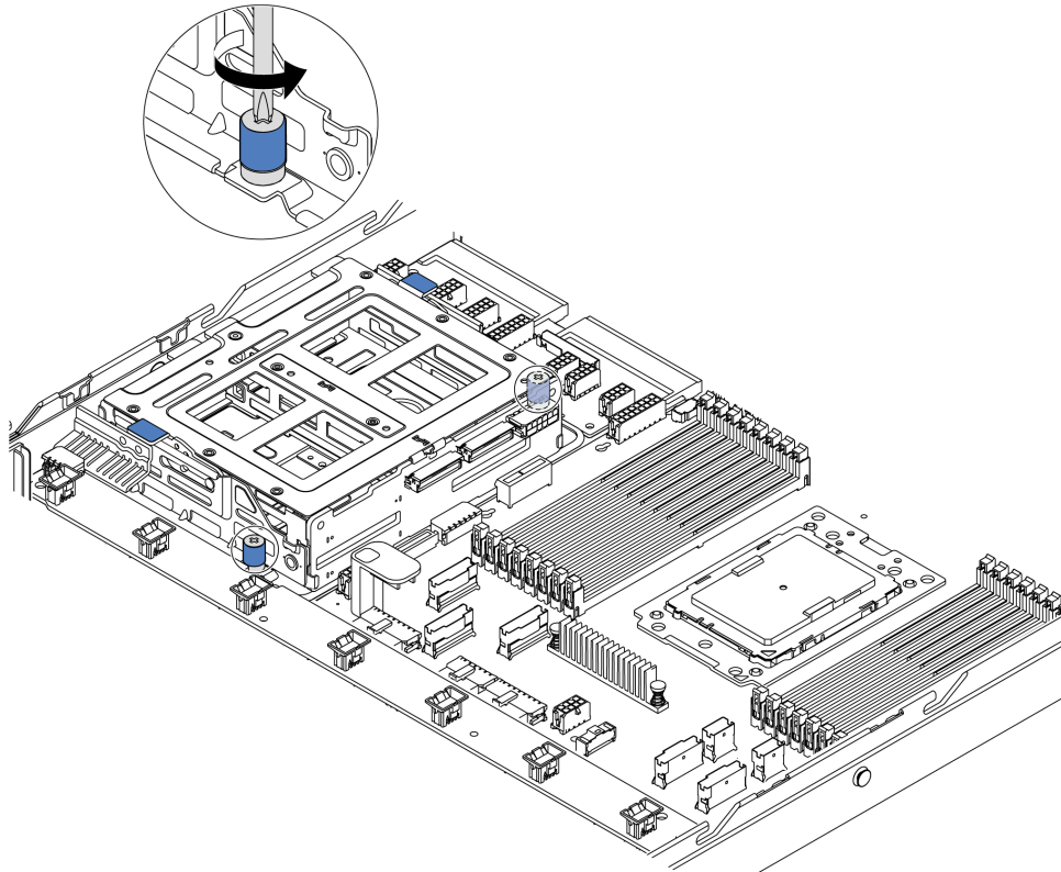
图 138. 卸下中间硬盘仓 - 1
