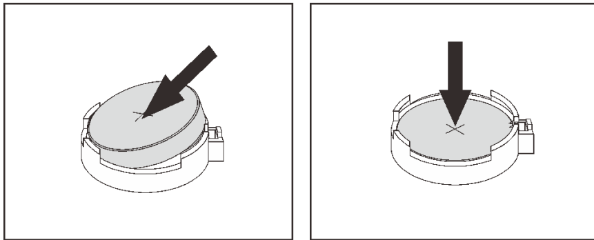
图 126. 安装 CMOS 电池
