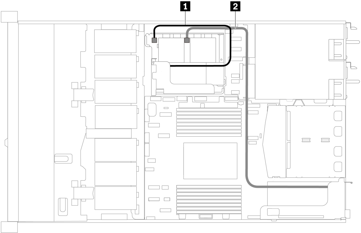
图 61. 配备两个超级电容器的服务器型号的线缆布放
