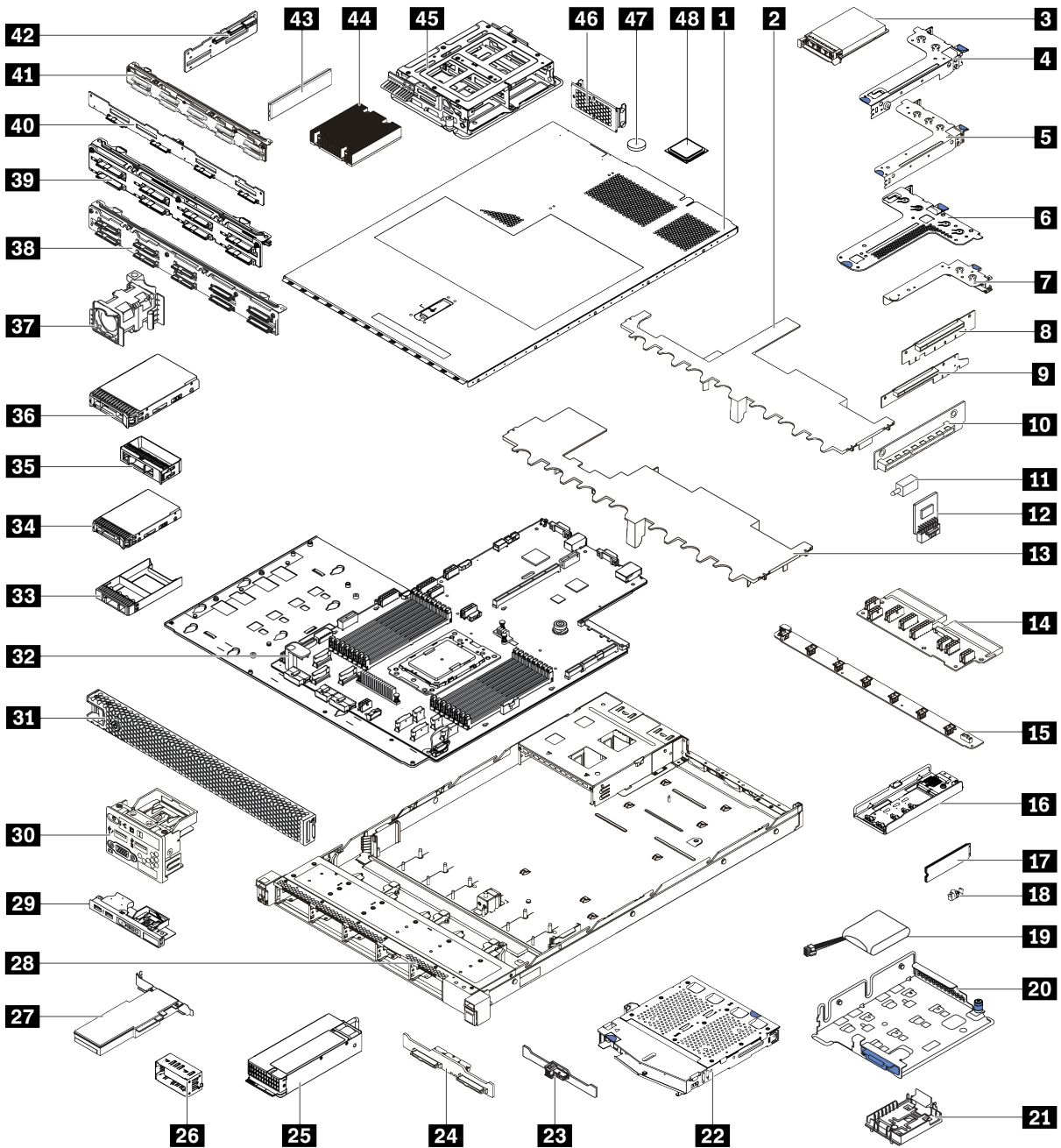
图 66. 服务器组件
