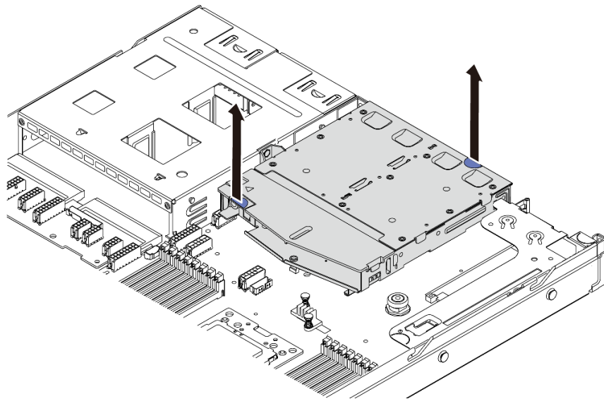
图 129. 卸下背面热插拔硬盘仓
