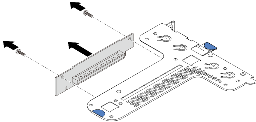
图 101. 卸下转接卡
