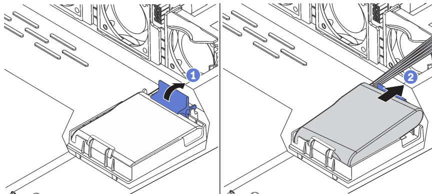
圖例 156. 卸下機箱上的 RAID 超級電容器模組
