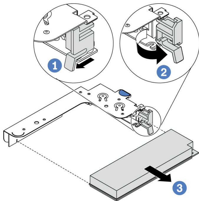
圖例 107. 內部擴充卡組件 (LP) 卸下
