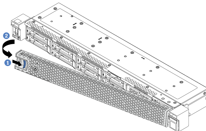
圖例 79. 卸下安全擋板
