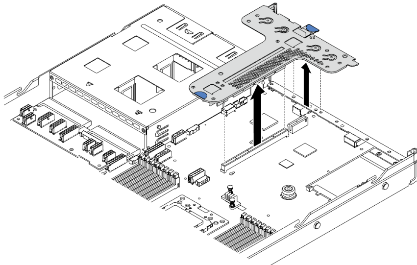
圖例 100. 卸下擴充卡組件
