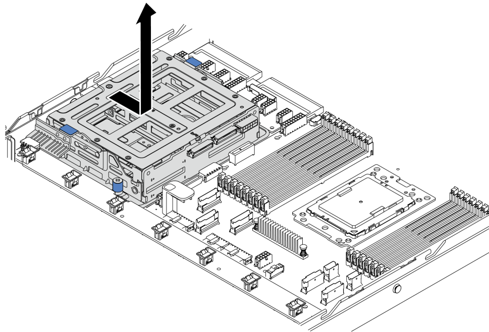
圖例 139. 卸下中間框架-2
