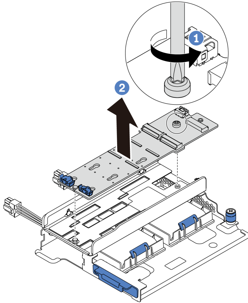
圖例 147. 卸下 M.2 配接卡
