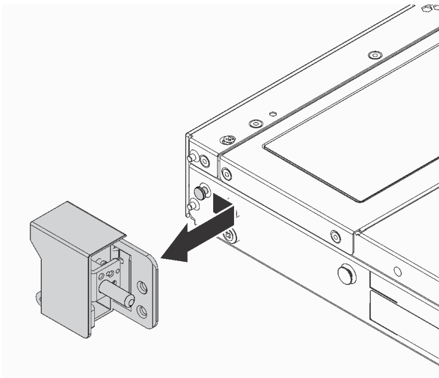
圖例 74. 機架門鎖拆卸
