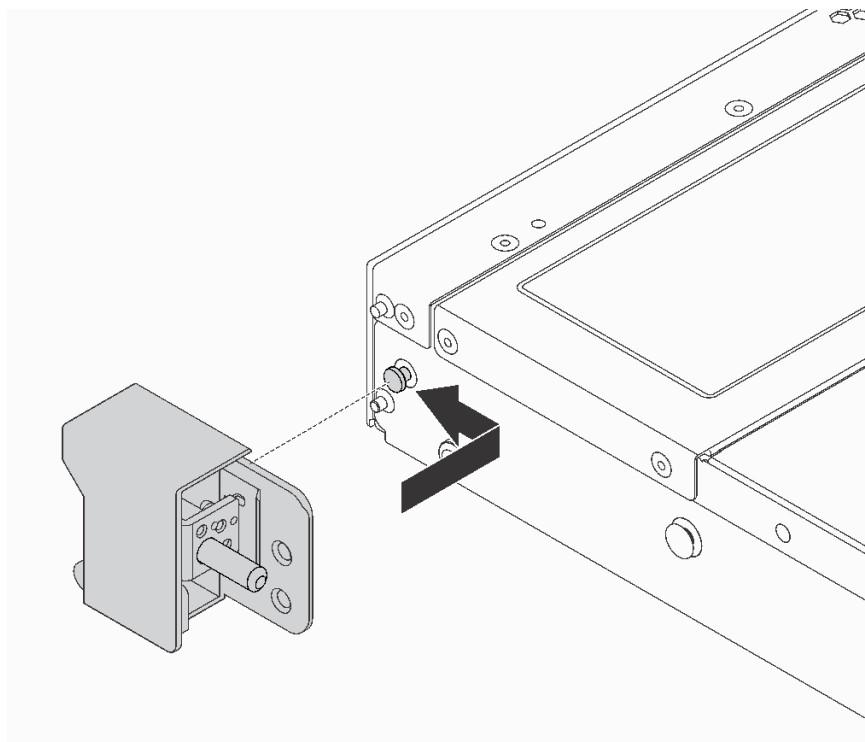
圖例 75. 機架門鎖安裝
