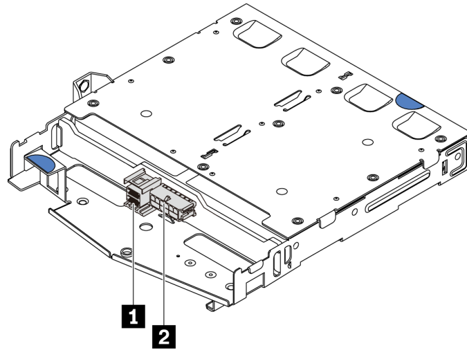
圖例 133. SAS/SATA 後方背板接頭
