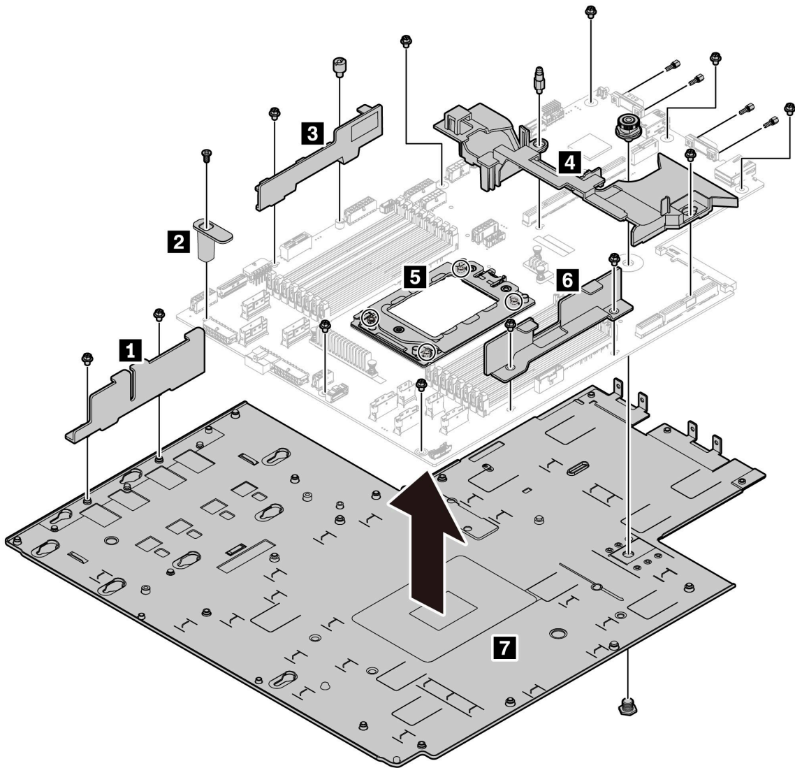
圖例 185. 拆卸主機板
