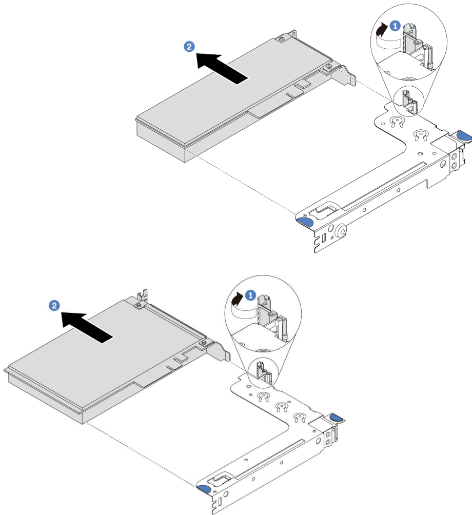
圖例 105. 擴充卡 1 組件 (LP/FHFL) 卸下
