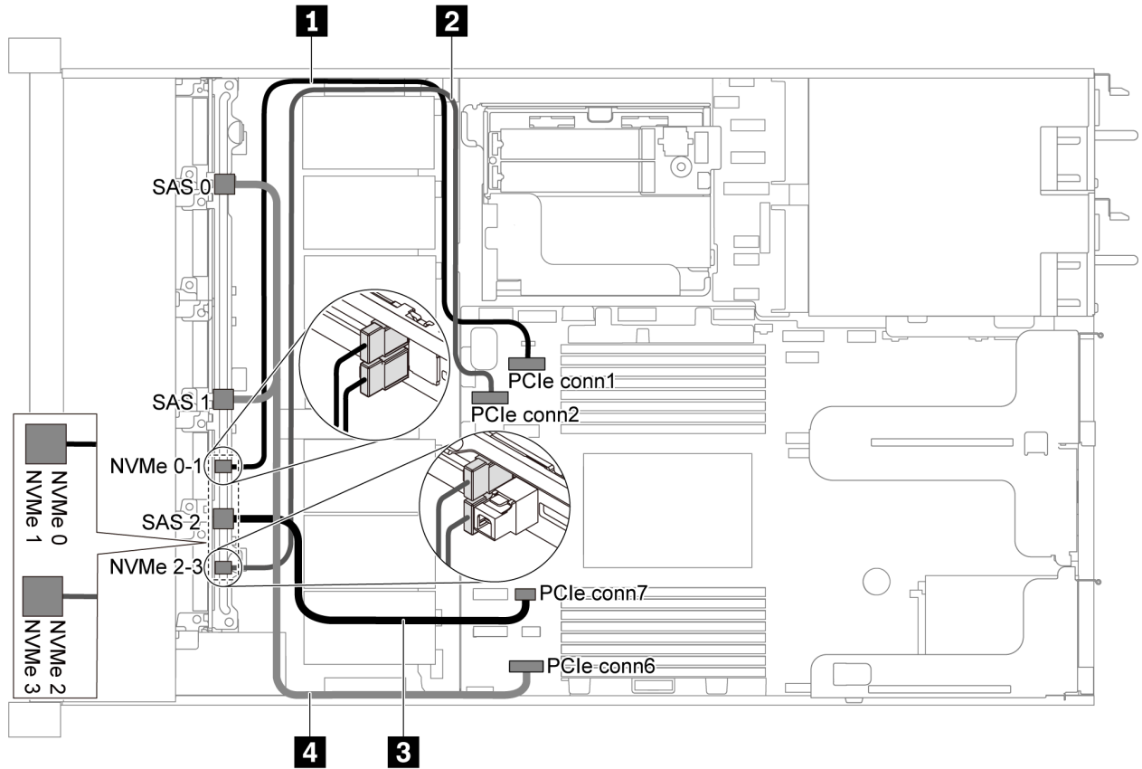
圖例 41. 配備六個 2.5 吋 SATA 硬碟及四個 2.5 吋 NVMe 硬碟之伺服器型號的纜線佈線
