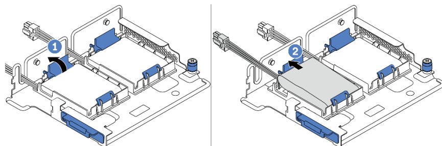
圖例 154. 卸下超級電容器模組
