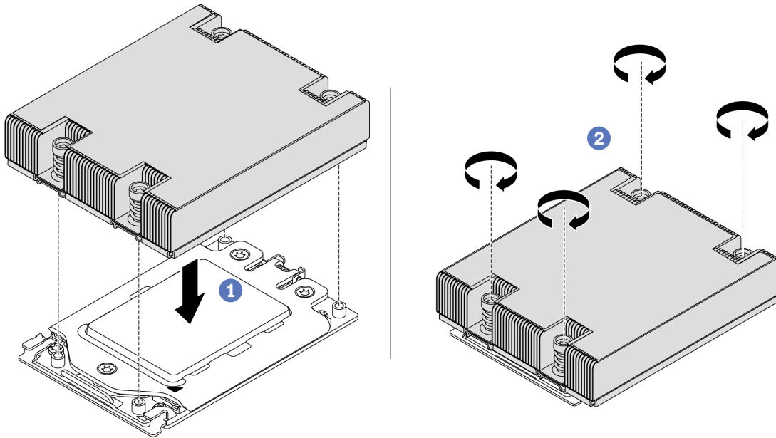
圖例 176. 安裝散熱槽
