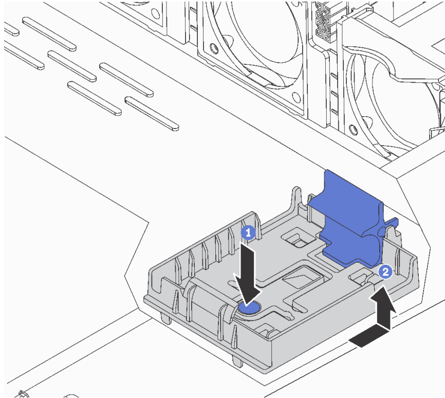
圖例 157. 卸下 RAID 超級電容器模組匣
