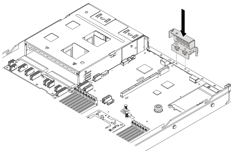
圖例 104. 後壁托架安裝
