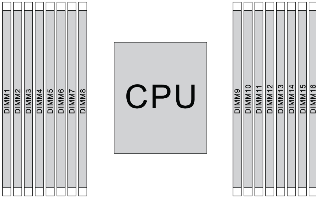
圖例 67. DIMM 位置
