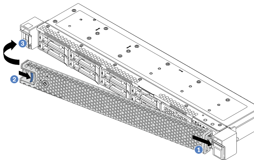
圖例 81. 安裝安全擋板
