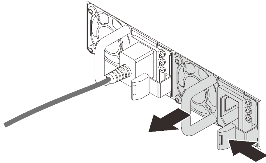
圖例 167. 卸下熱抽換電源供應器
