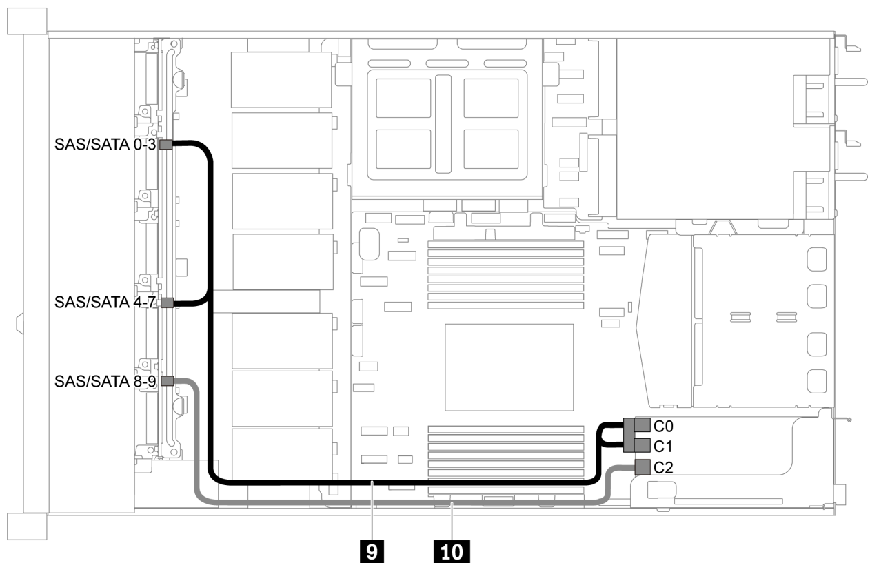
圖例 57. 配備十個 2.5 吋 SAS/SATA/NVMe 硬碟、背面 SAS/SATA 硬碟組件、中間 NVMe 硬碟組件及一個 16i RAID/HBA 配接卡-2 之伺服器型號的纜線佈線
