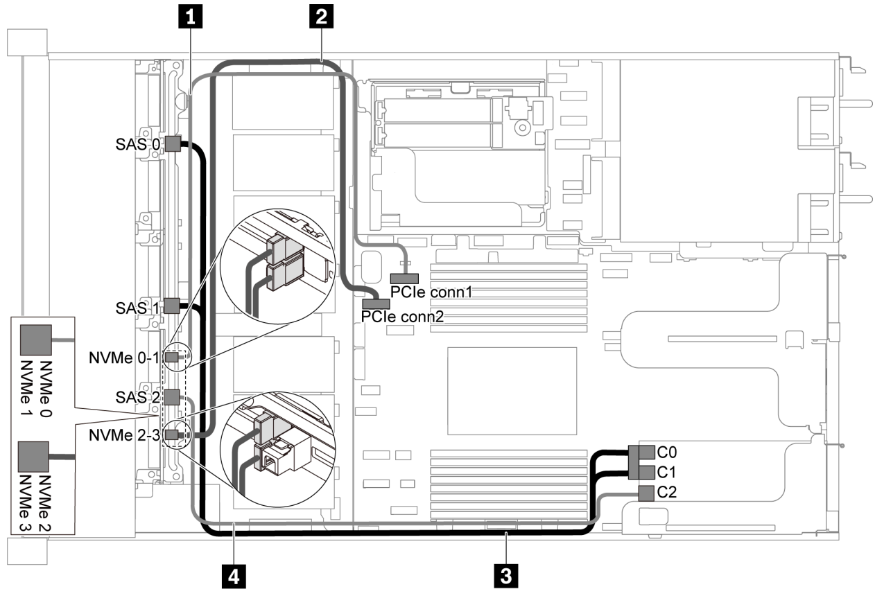
圖例 42. 配備六個 2.5 吋 SAS/SATA 硬碟、四個 2.5 吋 NVMe 硬碟和一個 16i RAID/HBA 配接卡之伺服器型號的纜線佈線
