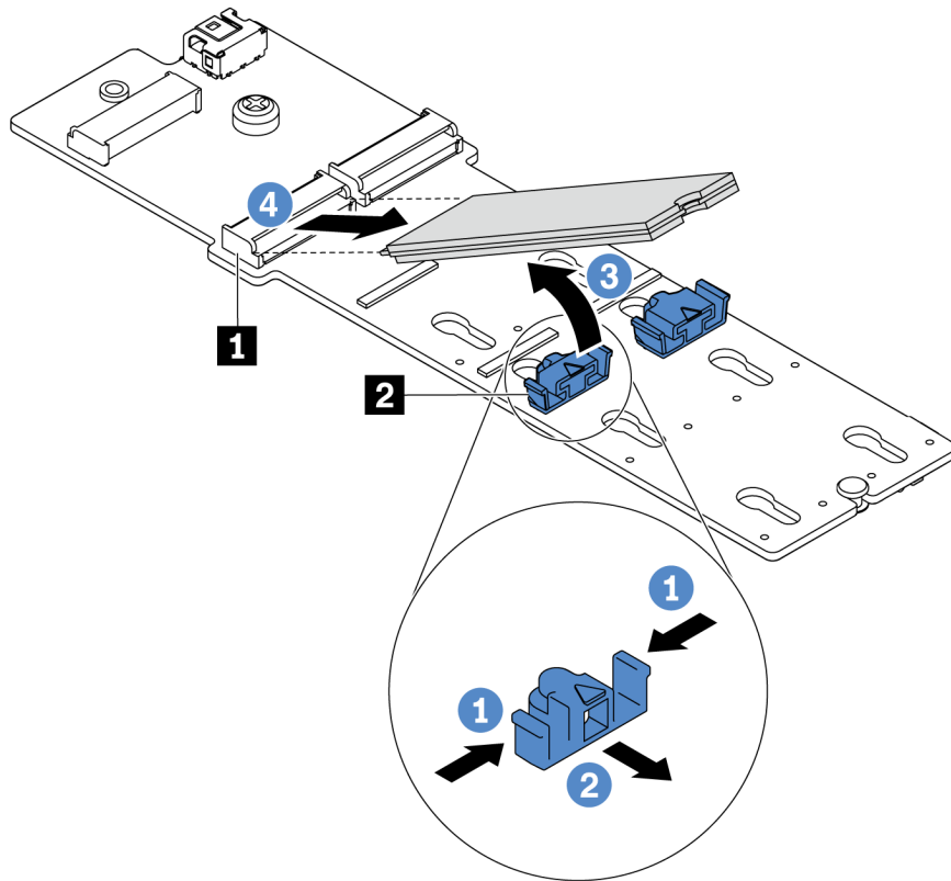
圖例 146. 卸下 M.2 硬碟
