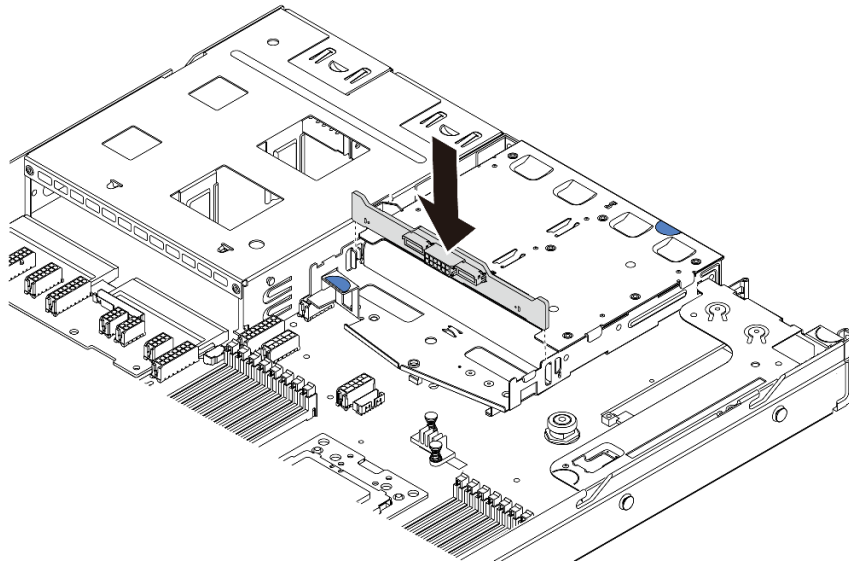
圖例 131. 安裝後方背板
