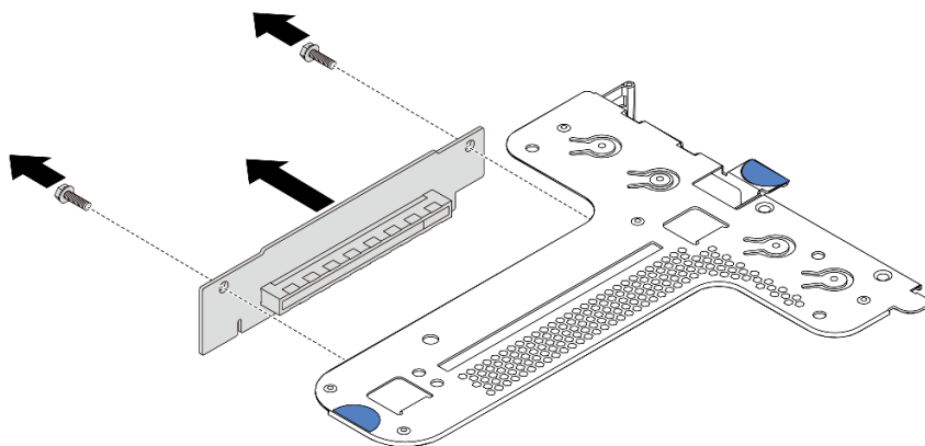
圖例 101. 卸下擴充卡
