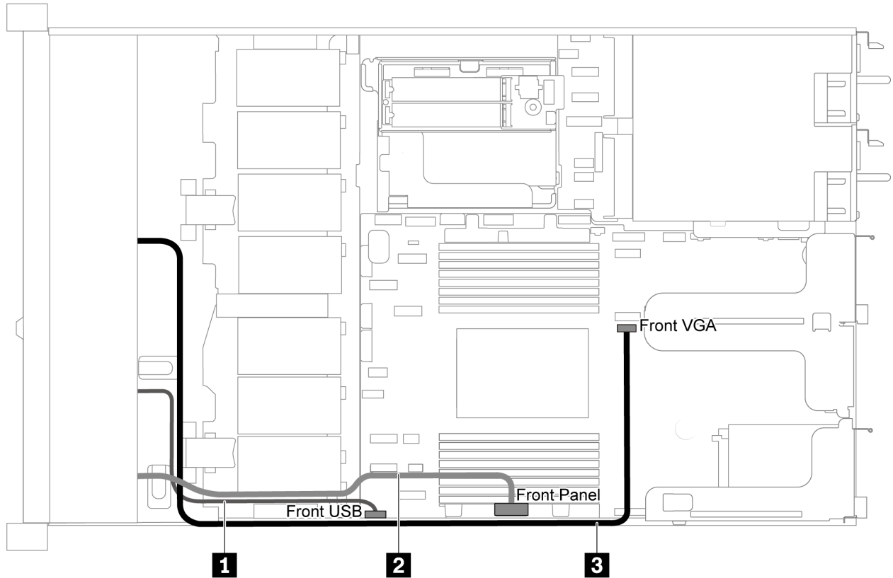
圖例 63. 配備四個 3.5 吋機槽之伺服器型號的 VGA/USB/前方面板接頭纜線佈線
