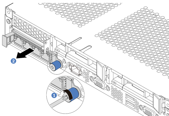
圖例 91. 卸下 OCP 3.0 乙太網路配接卡
