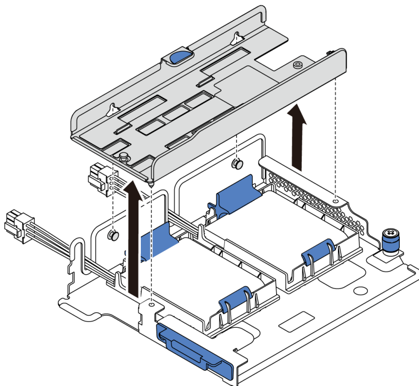
圖例 148. 卸下 M.2 配接卡托架
