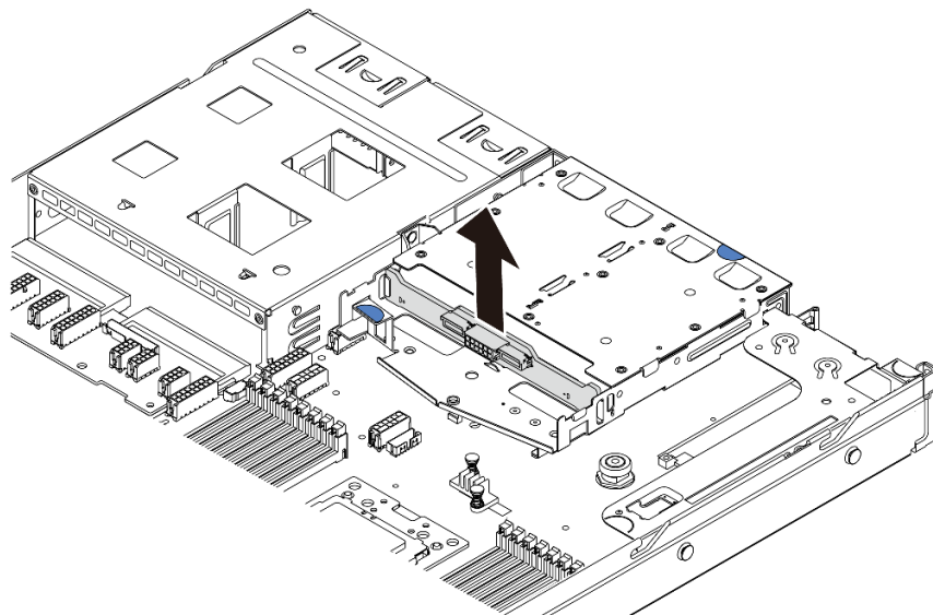
圖例 120. 卸下後方背板
