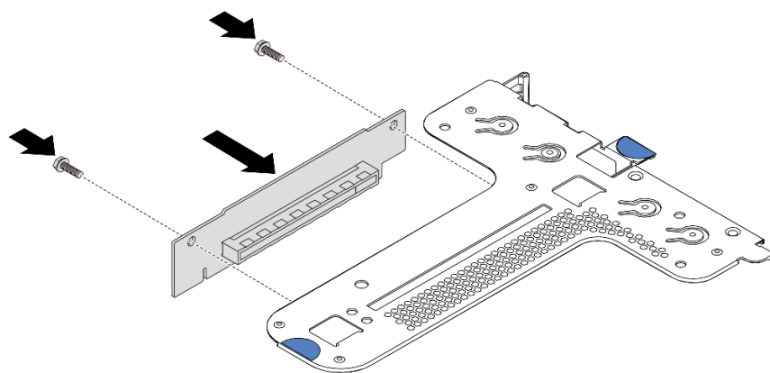
圖例 102. 擴充卡安裝
