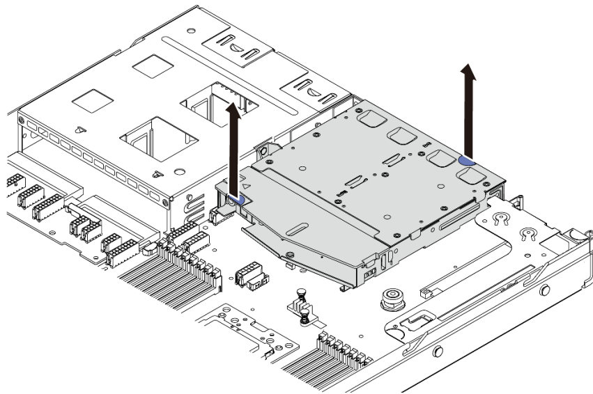
圖例 129. 卸下背面熱抽換硬碟框架
