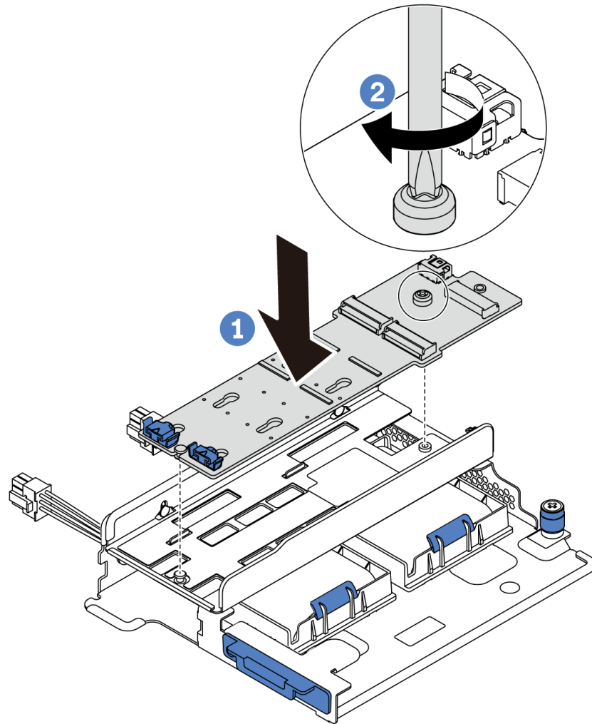
圖例 152. M.2 配接卡安裝
