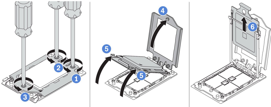
圖例 173. 卸下處理器
