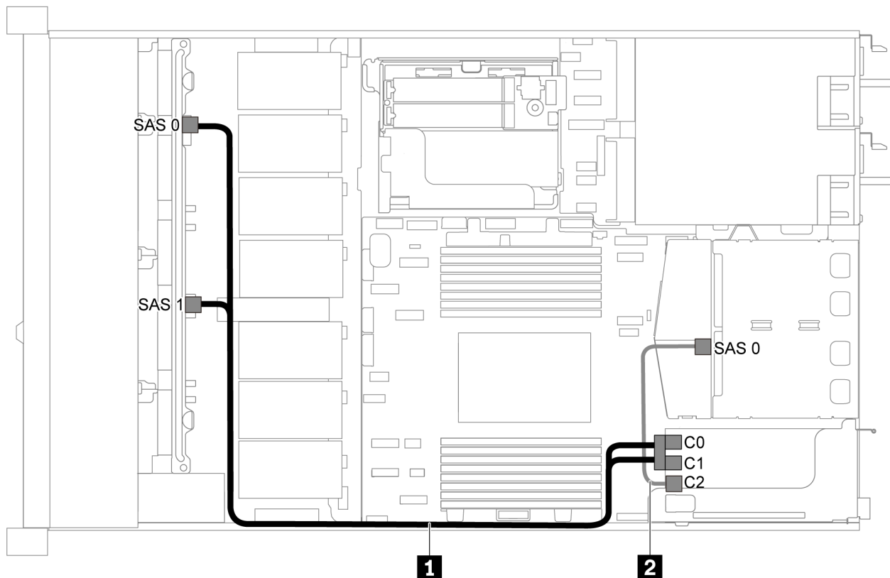
圖例 37. 配備八個 2.5 吋 SAS/SATA 硬碟、背面 SAS/SATA 硬碟組件及一個 16i RAID/HBA 配接卡之伺服器型號的纜線佈線
