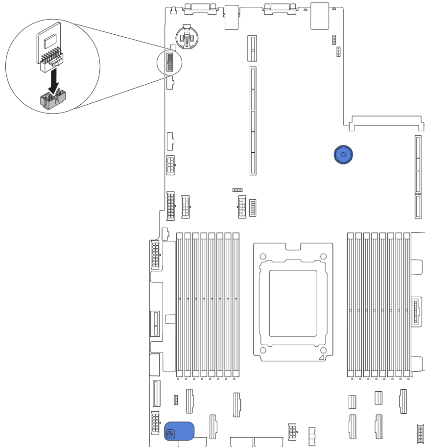
圖例 128. TPM 配接卡安裝
