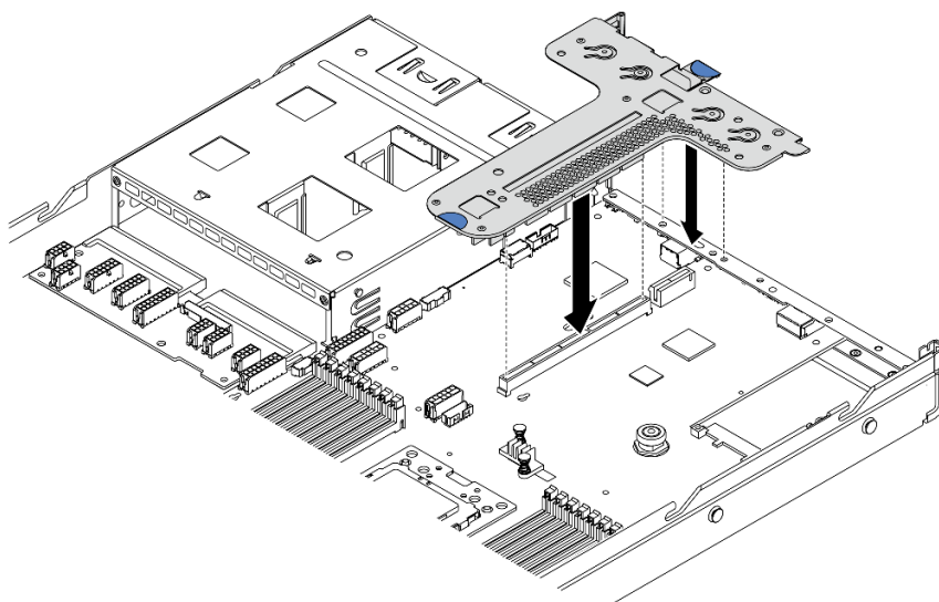
圖例 103. 安裝擴充卡組件
