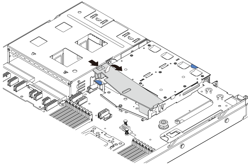
圖例 119. 卸下空氣擋板
