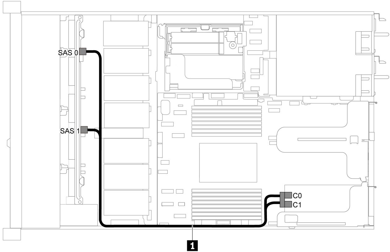
圖例 34. 配備八個 2.5 吋 SAS/SATA 硬碟及一個 8i RAID/HBA 配接卡的伺服器型號的纜線佈線
