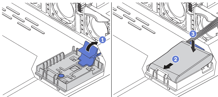
圖例 160. 安裝機箱上的 RAID 超級電容器模組
