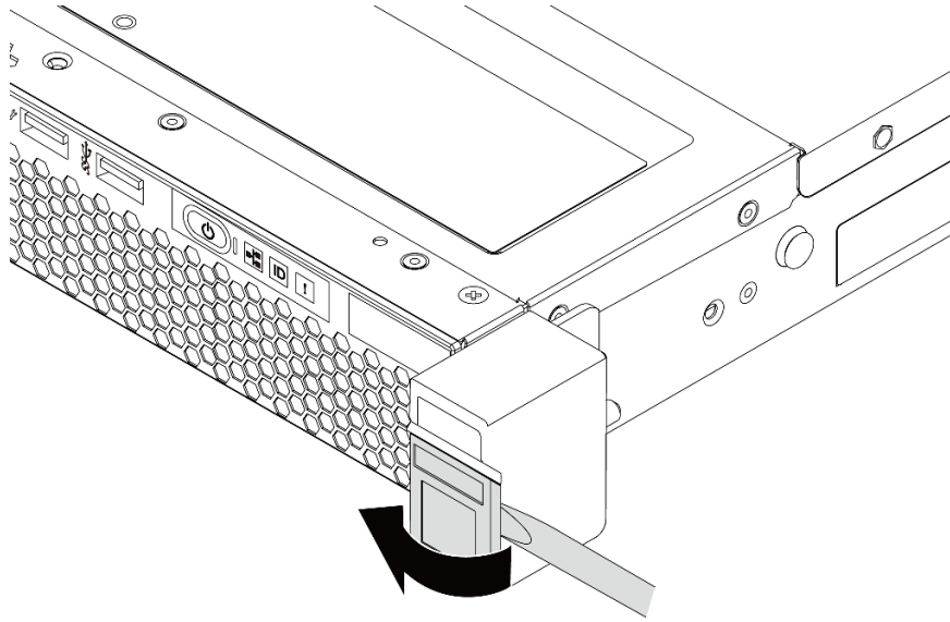
圖例 72. 卸下 ID 標籤板
