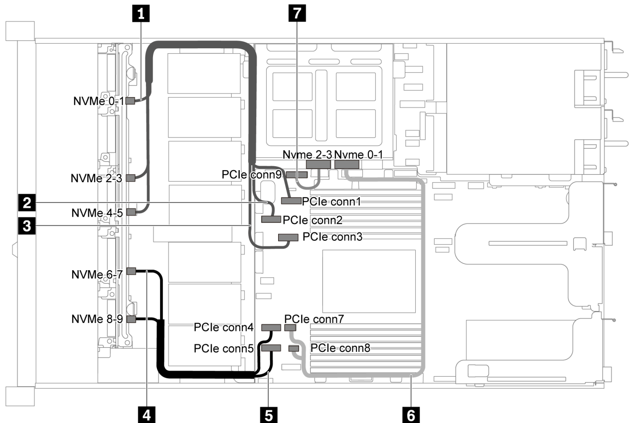
圖例 58. 配備十個 2.5 吋 SAS/SATA/NVMe 硬碟、中間 NVMe 硬碟組件及一個 16i RAID/HBA 配接卡-1 之伺服器型號的纜線佈線
