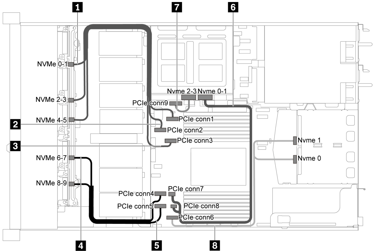
圖例 56. 配備十個 2.5 吋 SAS/SATA/NVMe 硬碟、背面 NVMe 硬碟組件、中間 NVMe 硬碟組件及一個 16i RAID/HBA 配接卡-1 之伺服器型號的纜線佈線
