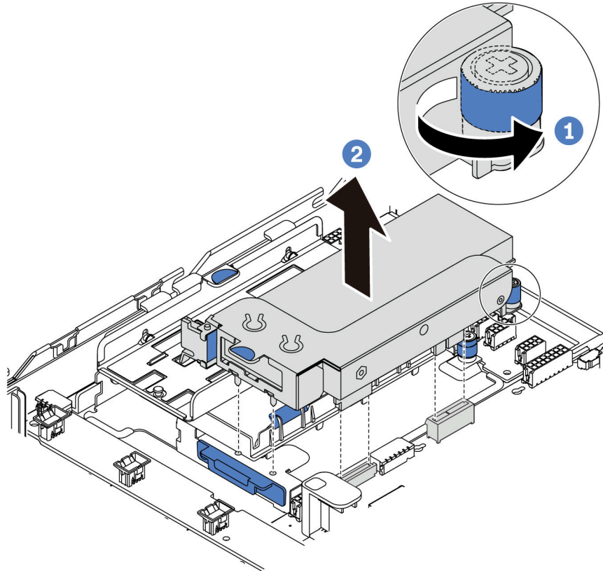
圖例 95. 卸下內部擴充卡組件
