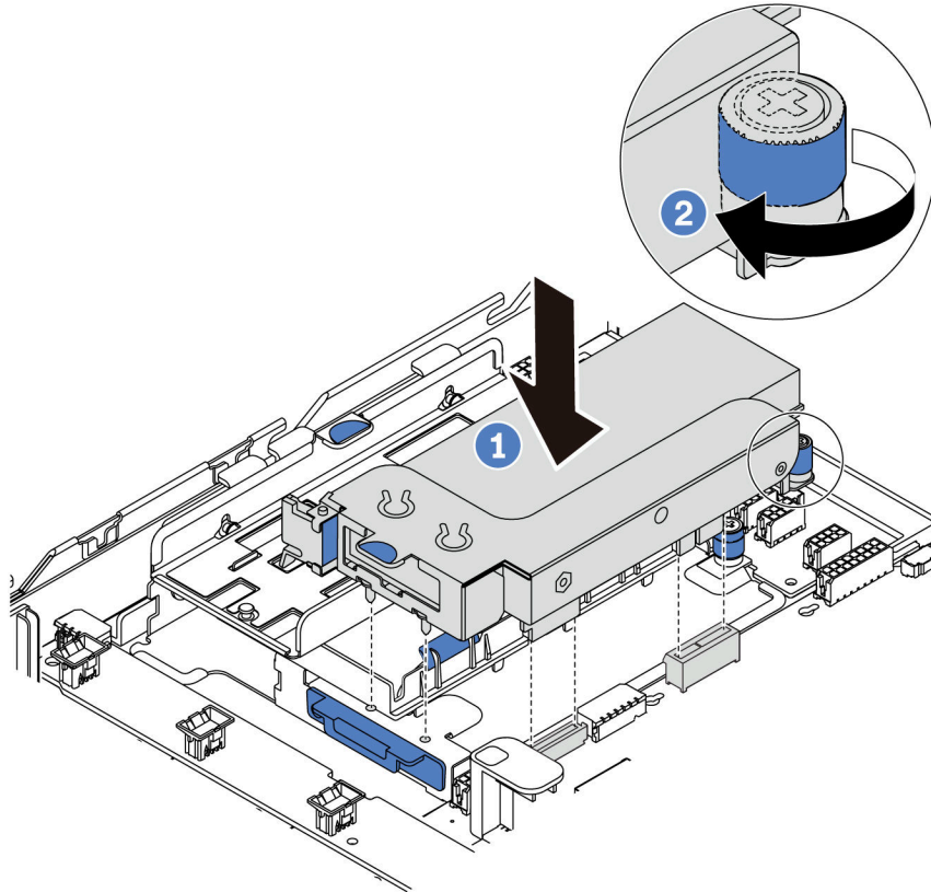
圖例 96. 內部擴充卡組件安裝
