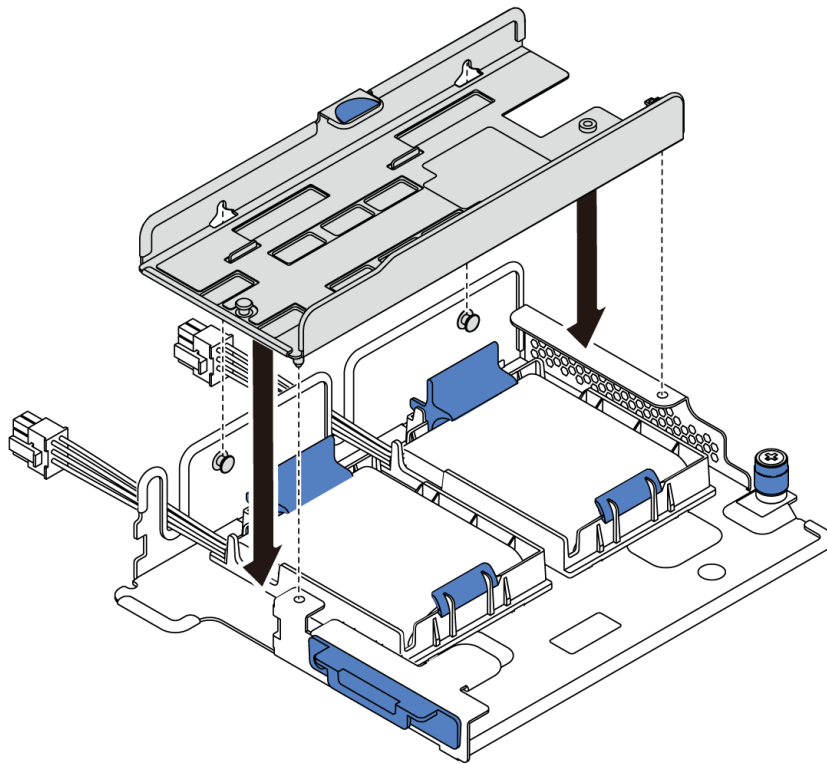
圖例 151. M.2 模組托架安裝
