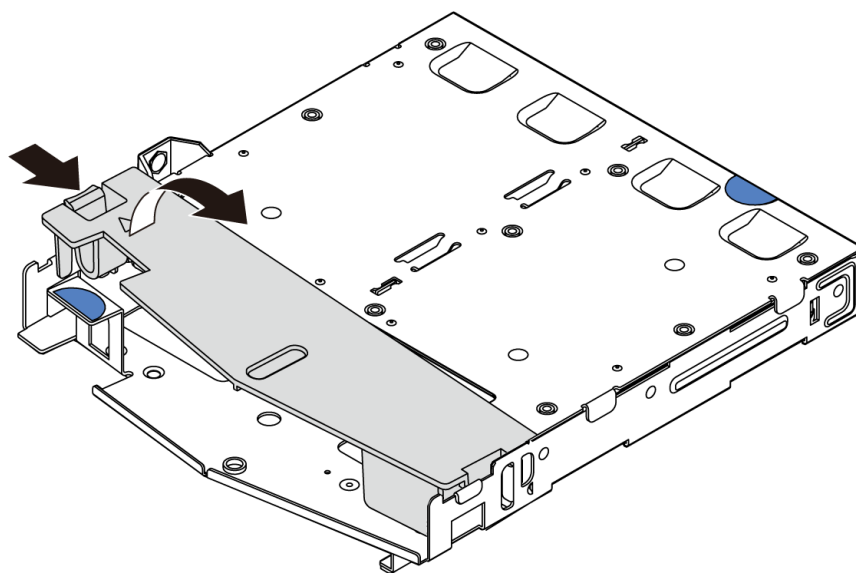
圖例 130. 卸下空氣擋板
