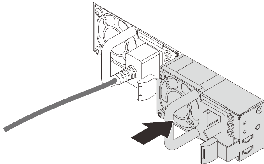
圖例 171. 安裝熱抽換電源供應器
