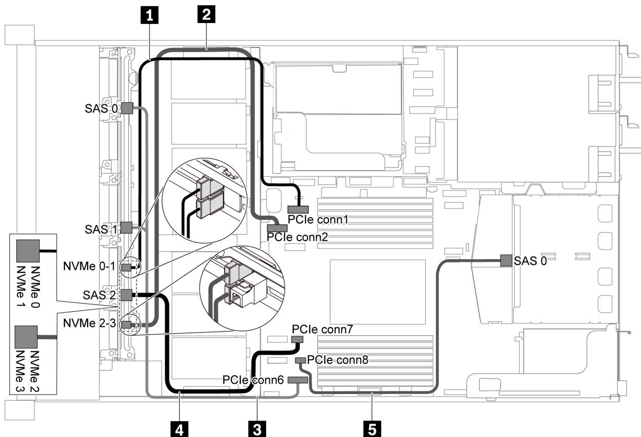
圖例 43. 配備六個 2.5 吋 SATA 硬碟、四個 2.5 吋 NVMe 硬碟及背面 SAS/SATA 硬碟組件之伺服器型號的纜線佈線
