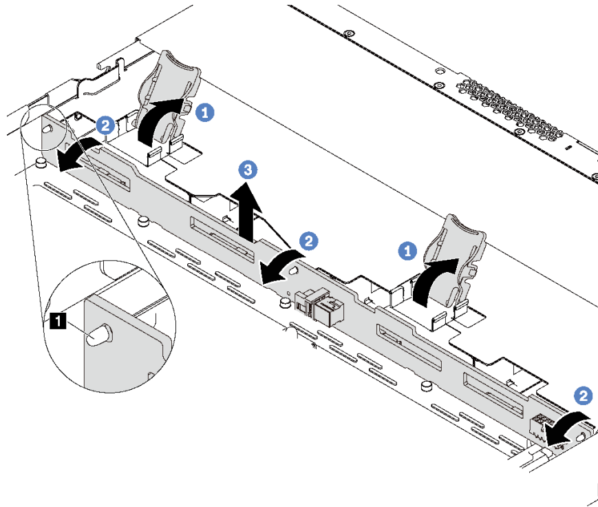
圖例 113. 卸下四個 3.5 吋熱抽換硬碟的背板
