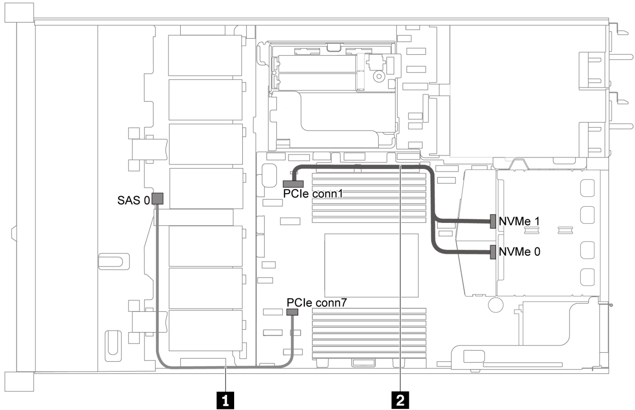
圖例 28. 配備四個 3.5 吋 SATA 硬碟及背面 NVMe 硬碟組件之伺服器型號的纜線佈線
