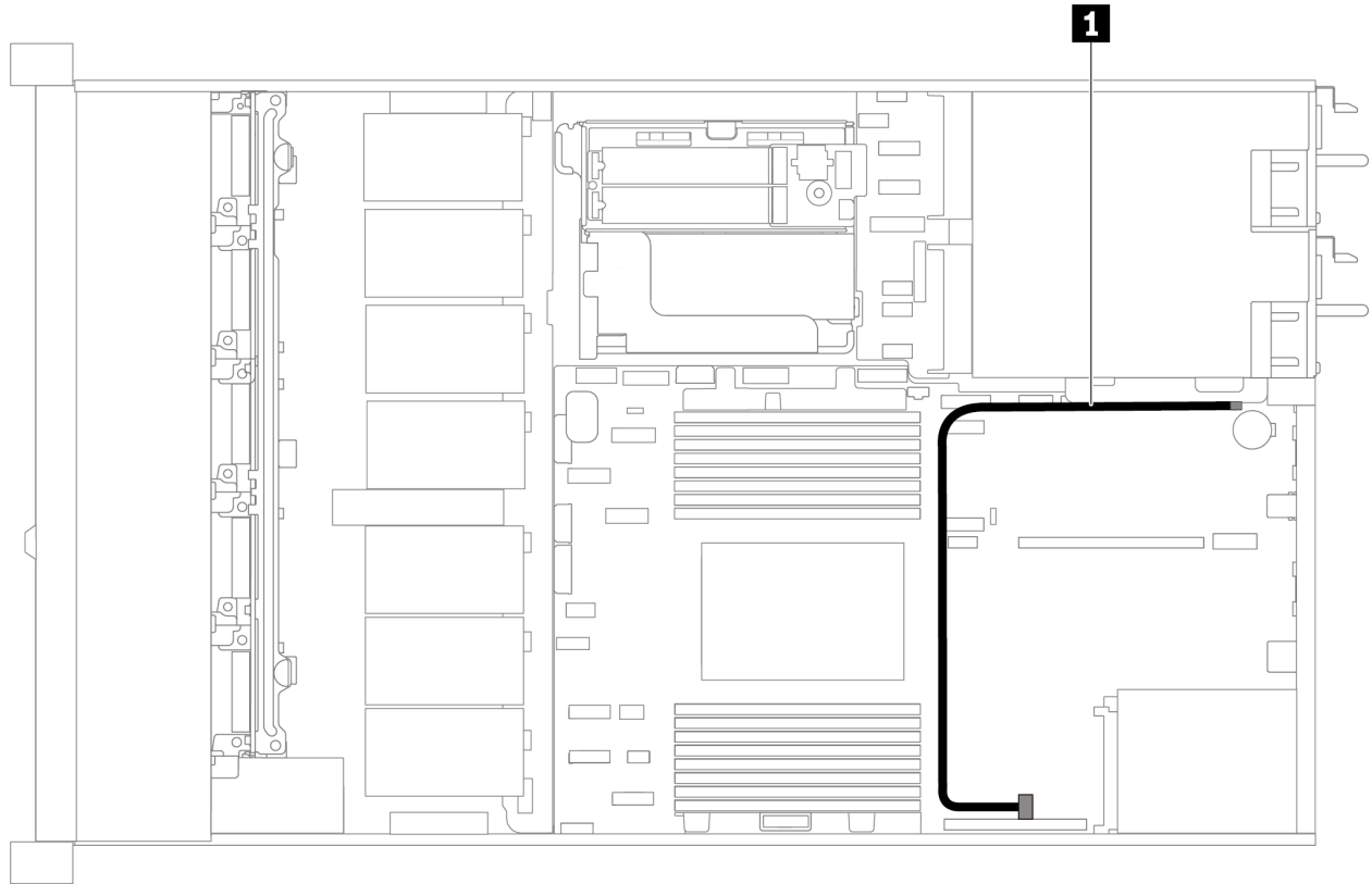
圖例 65. 配備入侵開關之伺服器型號的纜線佈線
