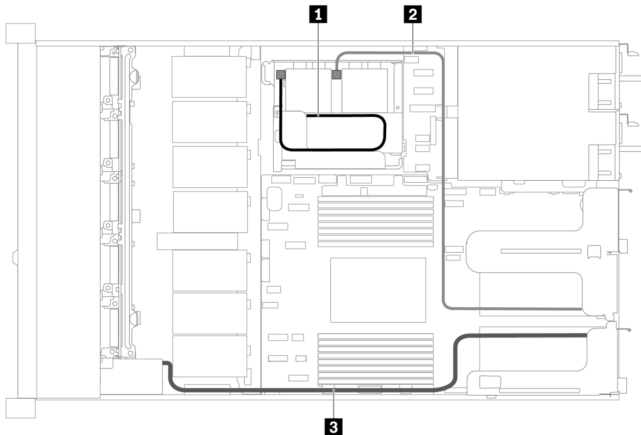
圖例 62. 配備三個超級電容器之伺服器型號的纜線佈線
