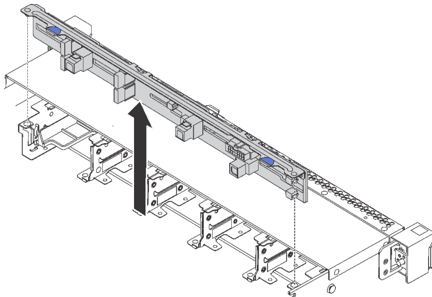
圖例 117. 卸下十個 2.5 吋熱抽換硬碟的背板
