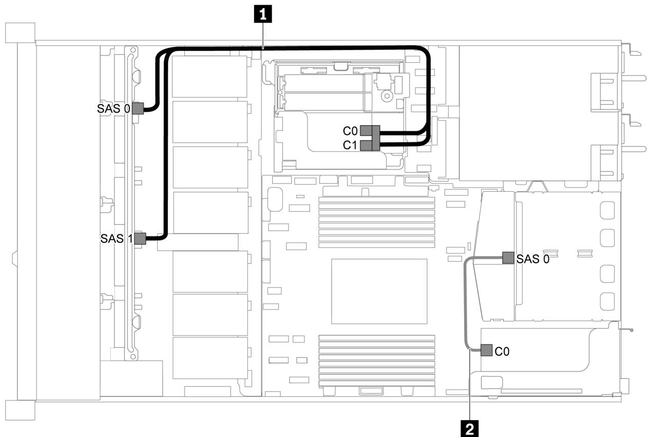
圖例 36. 配備八個 2.5 吋 SAS/SATA 硬碟、背面 SAS/SATA 硬碟組件及兩個 8i RAID/HBA 配接卡之伺服器型號的纜線佈線
