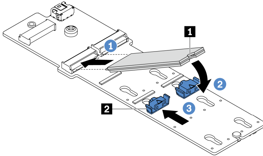
圖例 153. M.2 硬碟安裝
