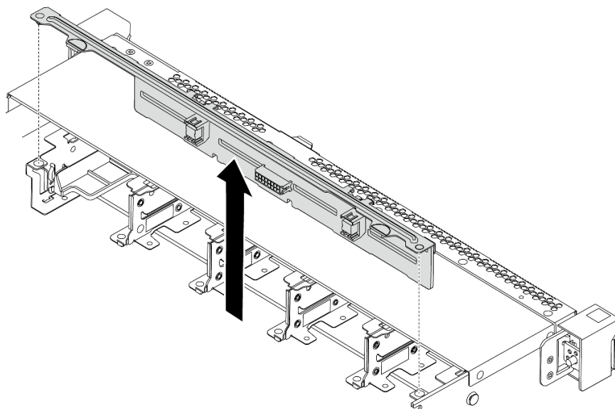
圖例 115. 卸下八個 2.5 吋熱抽換硬碟的背板
