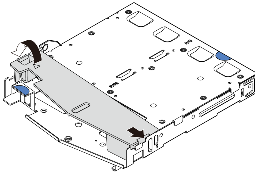
圖例 134. 安裝空氣擋板
