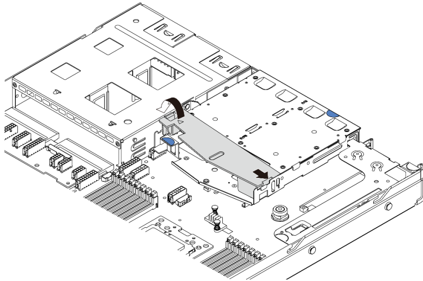
圖例 124. 安裝空氣擋板
