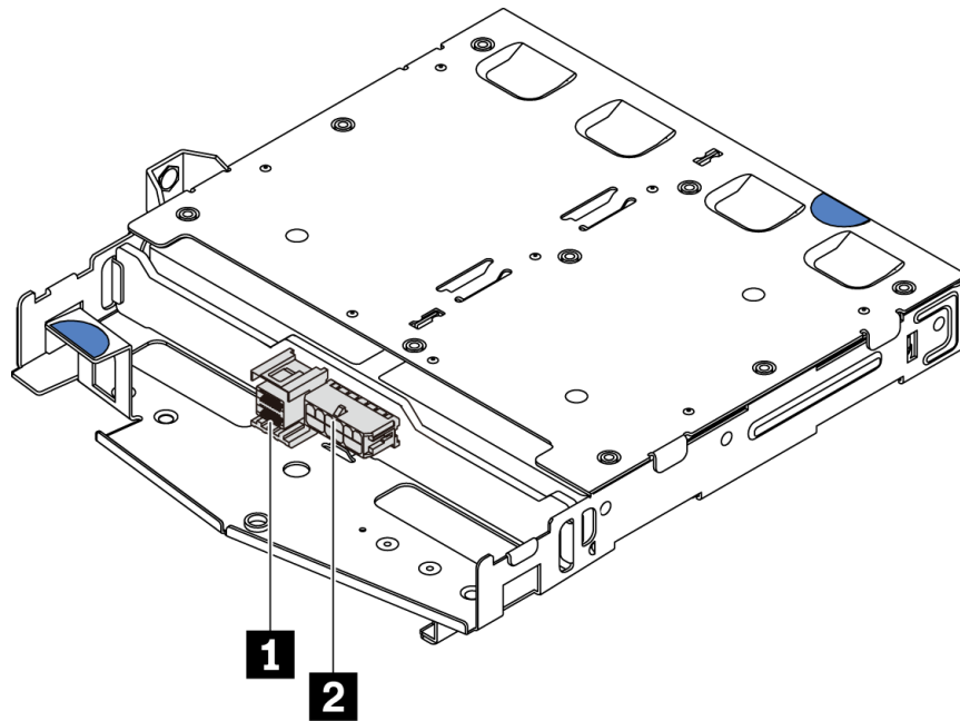
圖例 123. SAS/SATA 後方背板接頭
