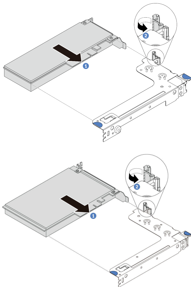
圖例 108. 擴充卡 1 組件 (LP/FHFL) 安裝
