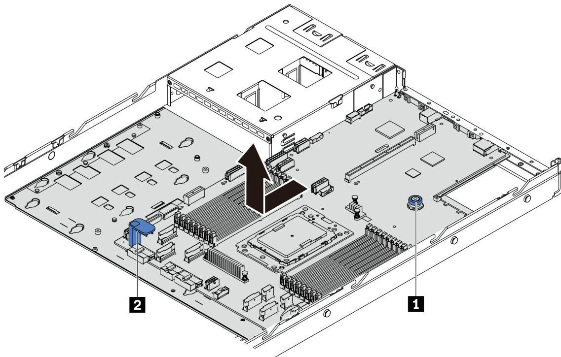
圖例 181. 卸下主機板
