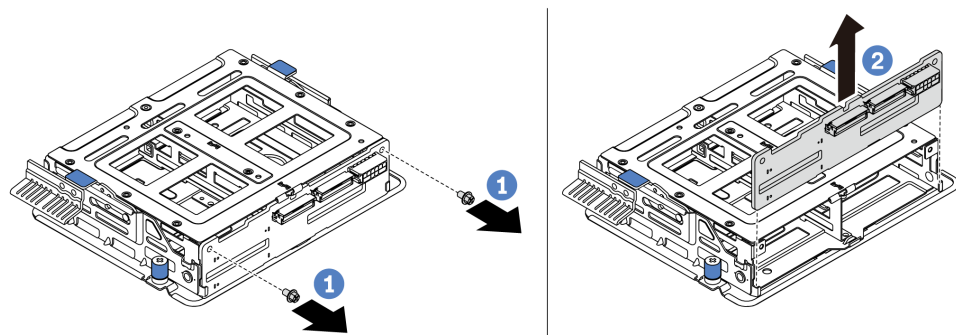
圖例 140. 卸下內部背板
