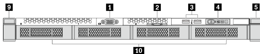
圖例 4. 未配備背板之伺服器型號的正面圖 (適用於四個 3.5 吋機槽)
