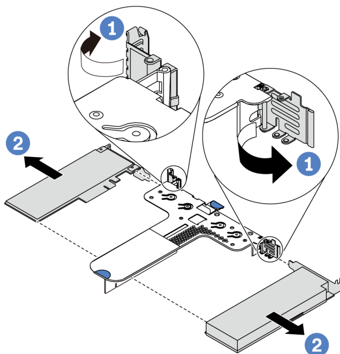
圖例 106. 擴充卡 2 組件 (LP/LP) 卸下
