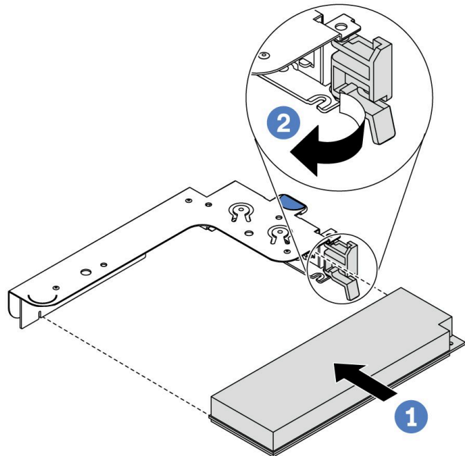
圖例 110. 內部擴充卡組件 (LP) 安裝
