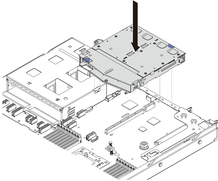
圖例 135. 安裝背面熱抽換硬碟框架
