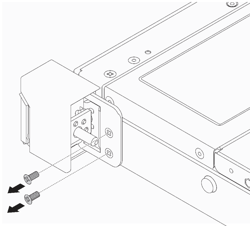
圖例 73. 卸下機架門鎖螺絲
