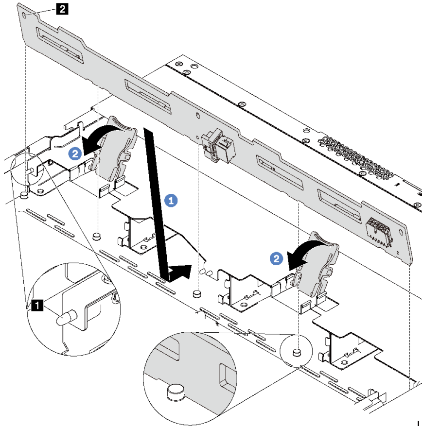
圖例 114. 安裝四個 3.5 吋熱抽換硬碟的背板
