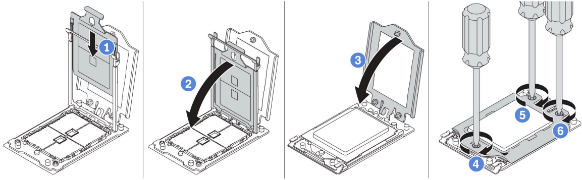
圖例 174. 安裝處理器
