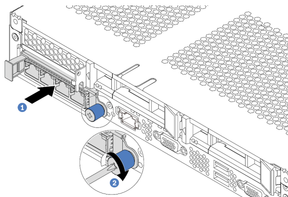
圖例 92. OCP 3.0 乙太網路配接卡安裝
