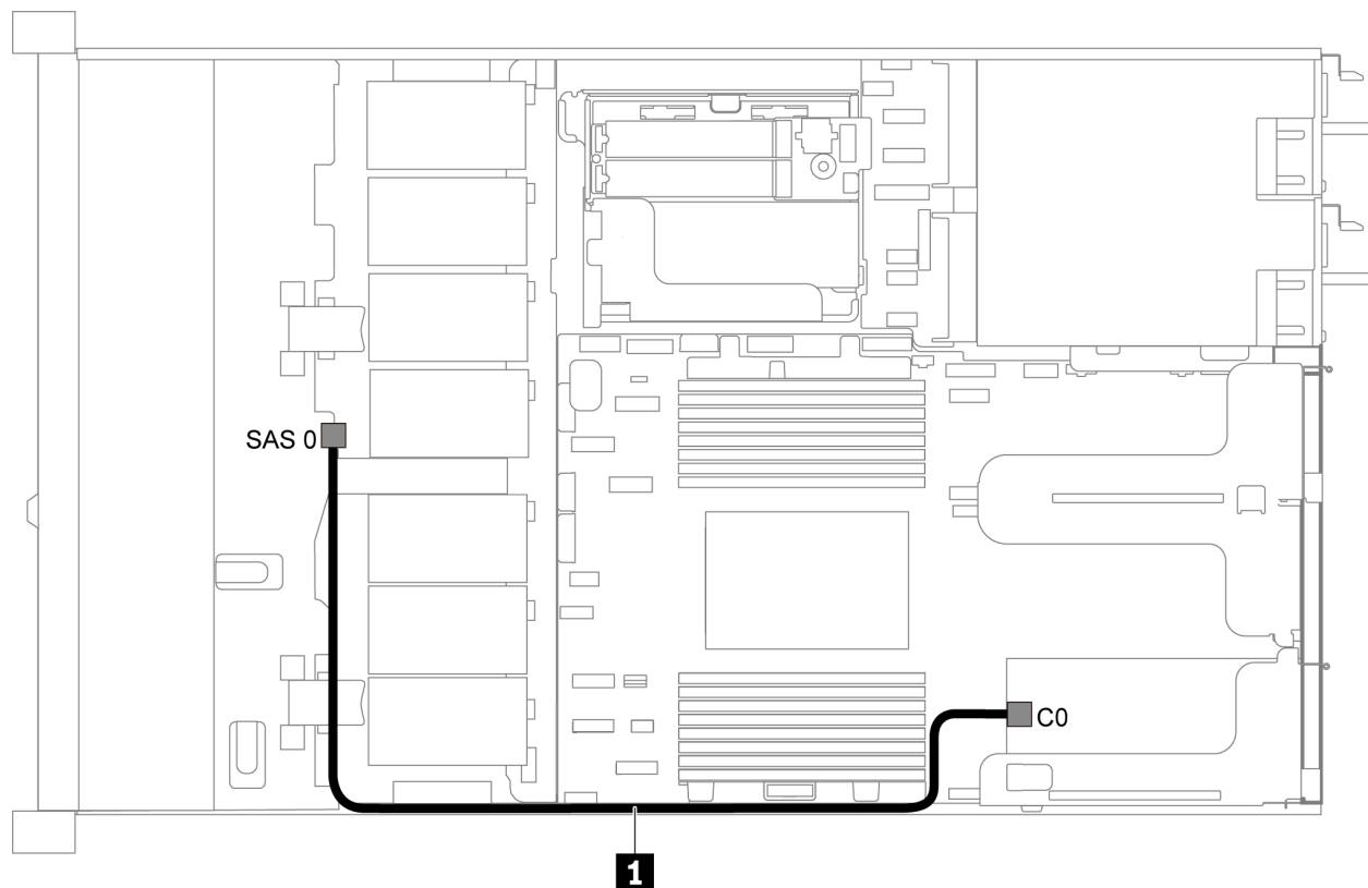
圖例 25. 配備四個 3.5 吋 SAS/SATA 硬碟及一個 8i RAID/HBA 配接卡之伺服器型號的纜線佈線
