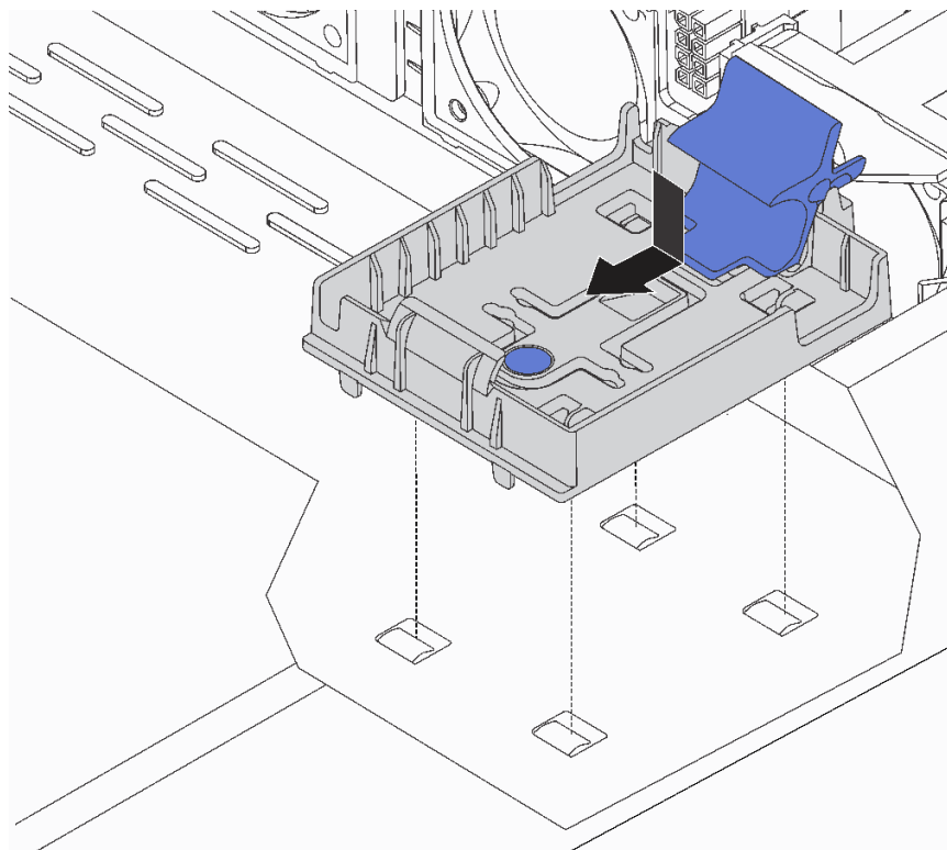
圖例 159. 安裝 RAID 超級電容器模組匣
