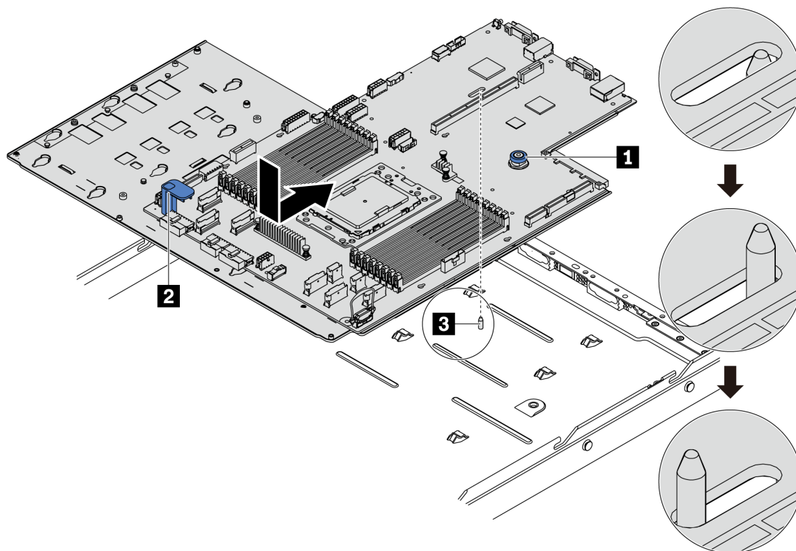
圖例 182. 安裝主機板
