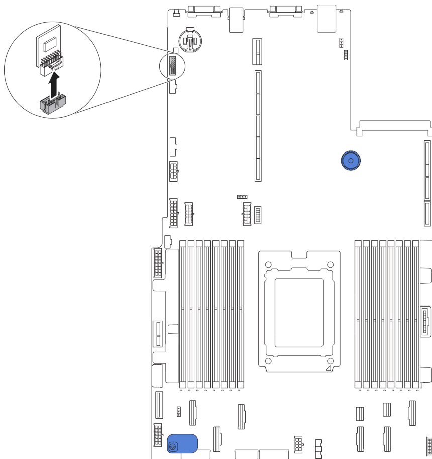
圖例 127. 卸下 TPM 配接卡
