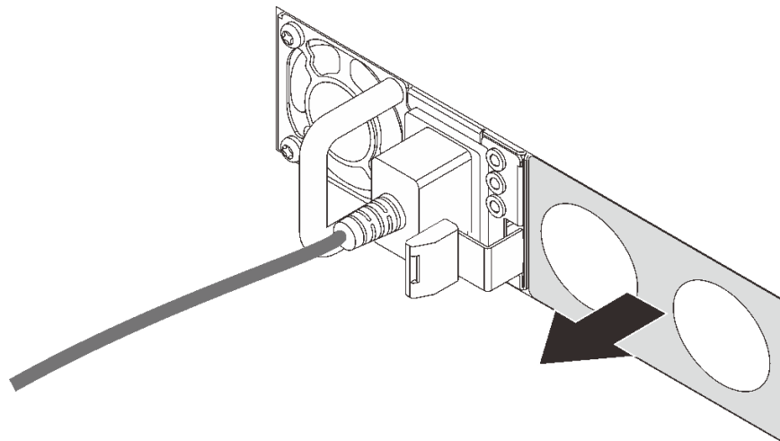
圖例 170. 卸下熱抽換電源供應器填充板
