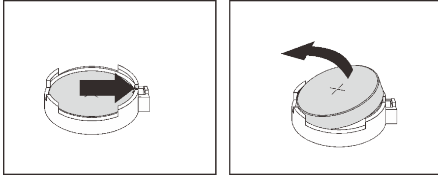
圖例 125. 卸下 CMOS 電池
