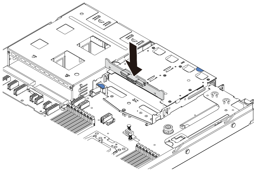
圖例 121. 安裝後方背板
