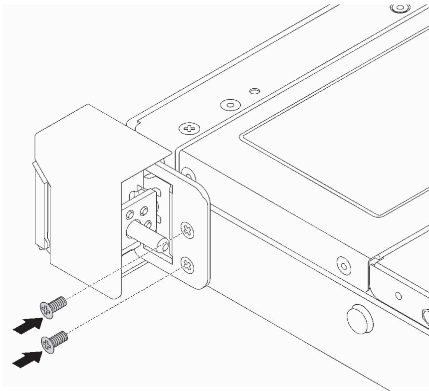
圖例 76. 機架門鎖螺絲安裝
