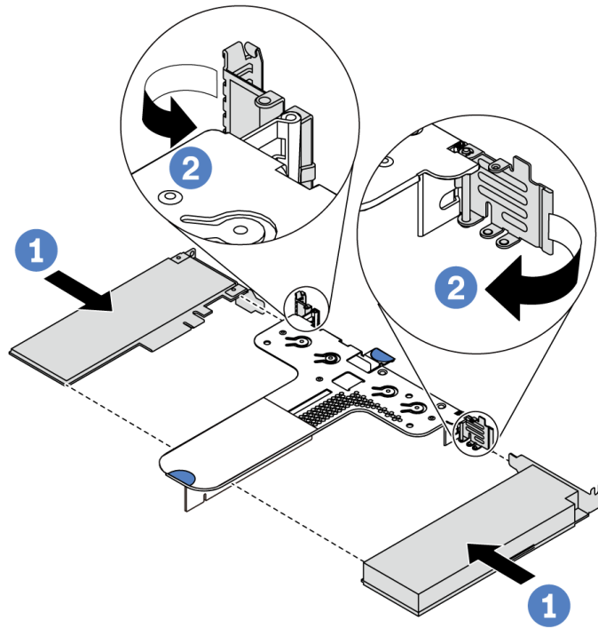
圖例 109. 擴充卡 2 組件 (LP+LP) 安裝
