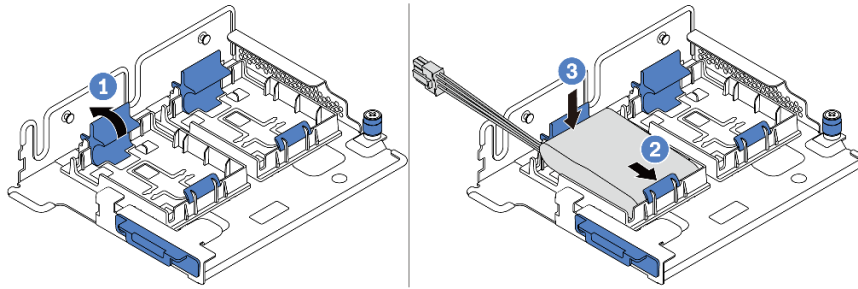
圖例 155. 超級電容器模組安裝
