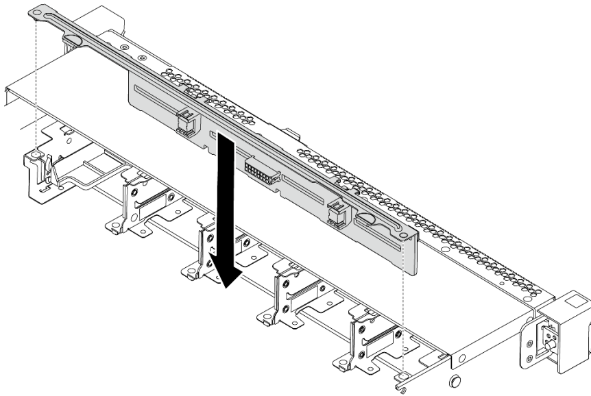
圖例 116. 安裝八個 2.5 吋熱抽換硬碟的背板
