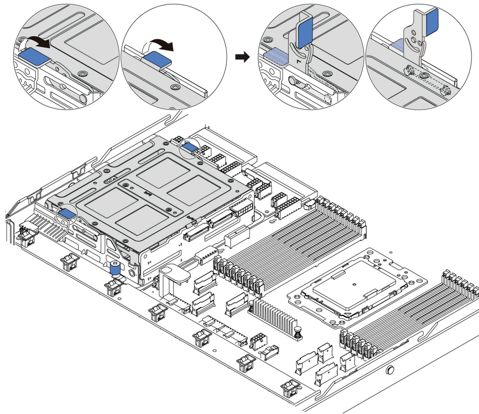
圖例 136. 卸下內部硬碟-1
