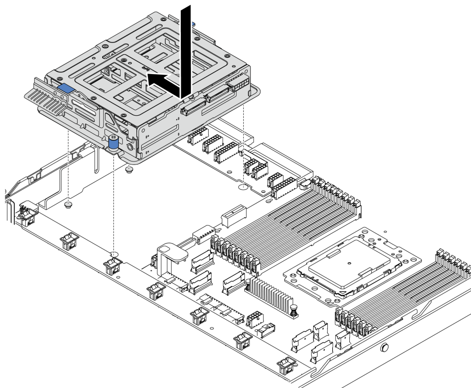
圖例 142. 中間框架安裝-1
