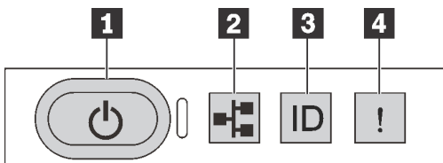
그림 17. 앞면 오퍼레이터 패널
