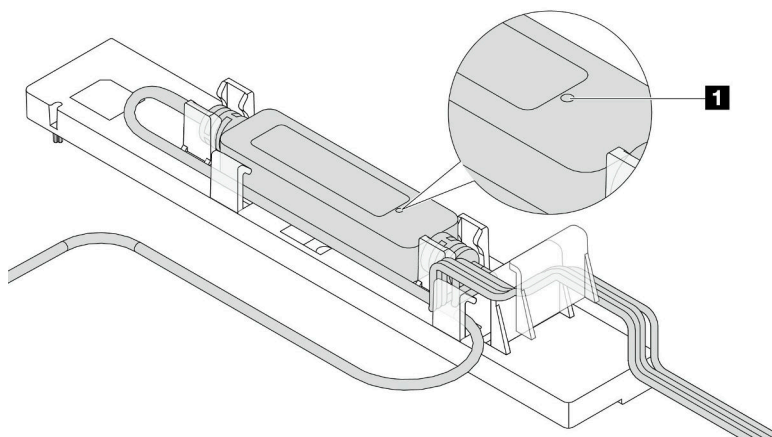
그림 24. 누수 감지 LED
