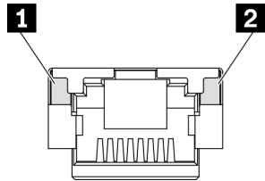
그림 23. XCC 시스템 관리 포트 LED
