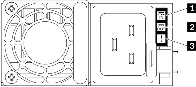
그림 21. 전원 공급 장치 LED
