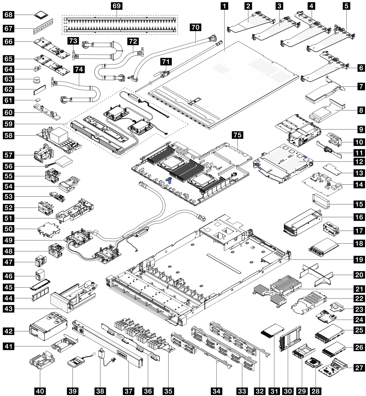
그림 25. 서버 구성 요소
