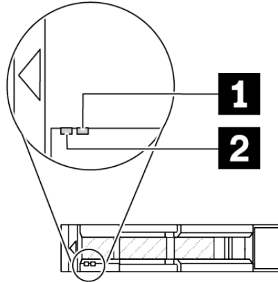
그림 18. 하드 디스크 드라이브 또는 솔리드 스테이트 드라이브의 LED
