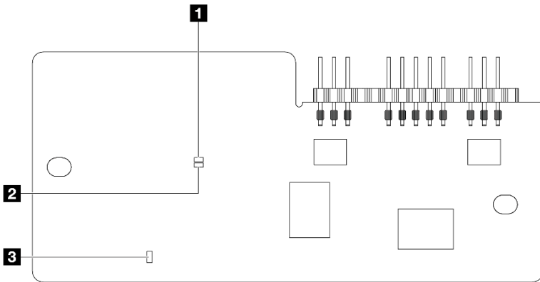
그림 20. 펌웨어 및 RoT 보안 모듈의 LED
