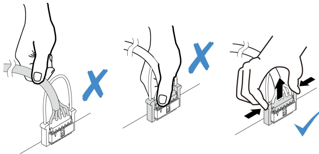
그림 124. 직렬 포트 케이블 분리
