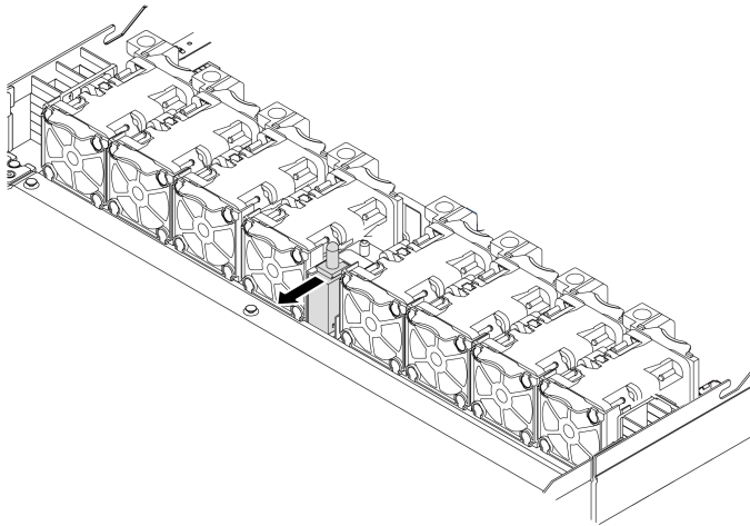
그림 81. 침입 스위치 제거
