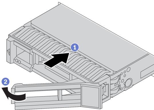
그림 55. 핫 스왑 드라이브 설치
