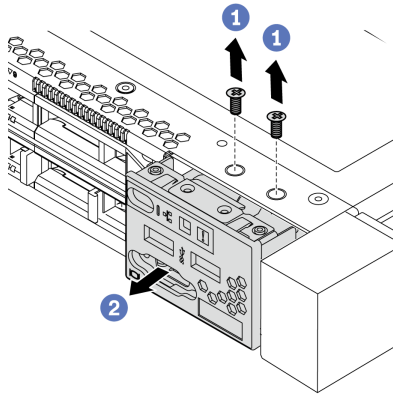
그림 45. 앞면 입/출력 어셈블리 제거
