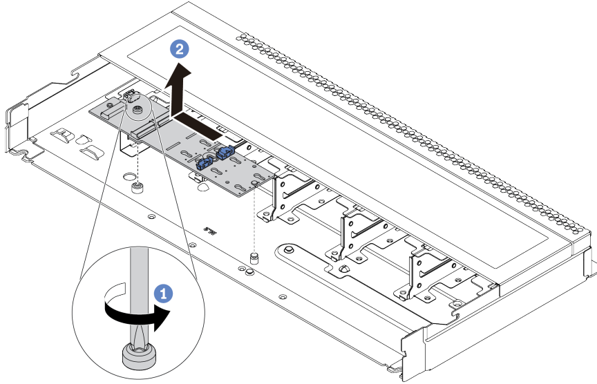
그림 86. M.2 모듈 제거
