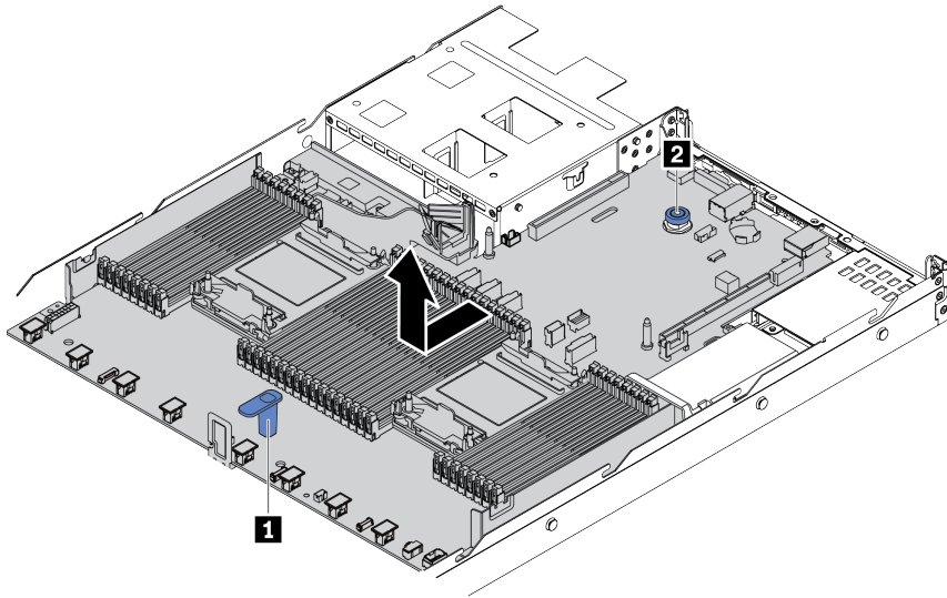
그림 137. 시스템 보드 제거
