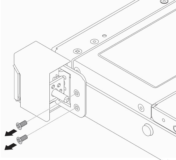
그림 98. 랙 래치 나사 제거
