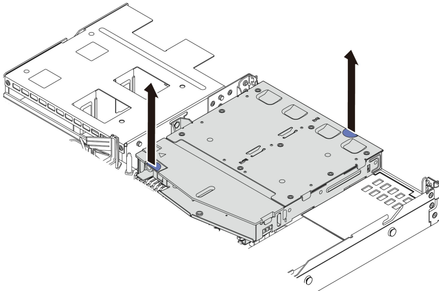
그림 68. 핫 스왑 뒷면 드라이브 케이스 제거
