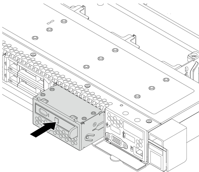
그림 51. 진단 패널 어셈블리 설치
