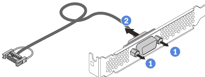
그림 125. 직렬 포트 모듈 분해
