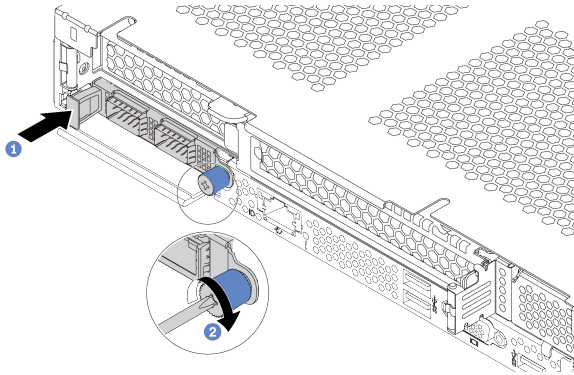
그림 94. OCP 3.0 이더넷 어댑터 설치
