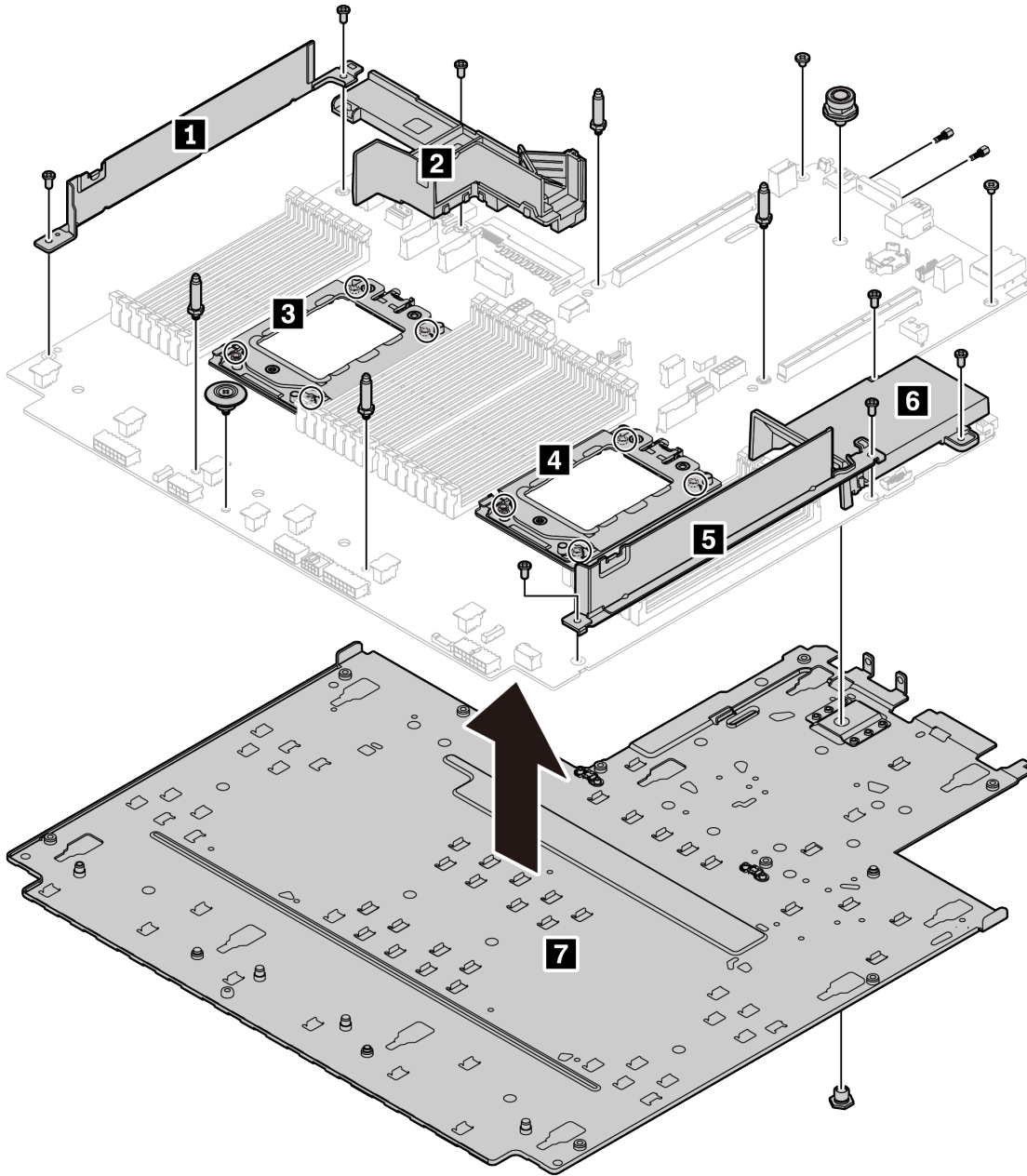
그림 140. 시스템 보드 분해
