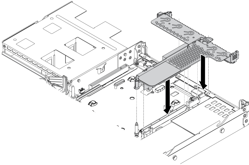
그림 116. 라이저 어셈블리 설치
