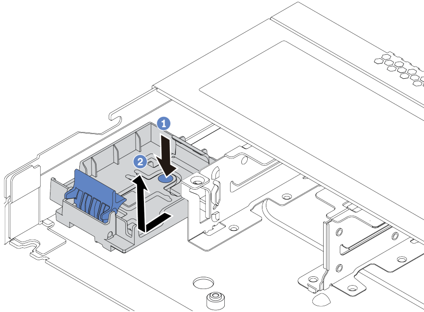
그림 104. RAID 슈퍼 커패시터 모듈 홀더 제거
