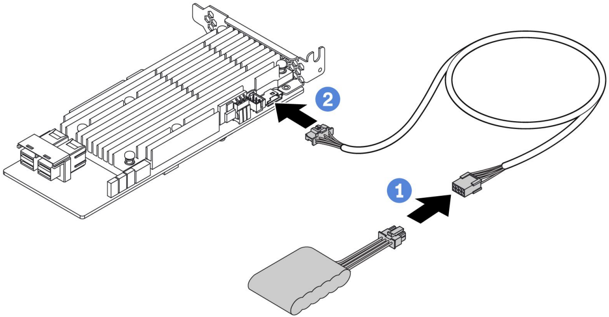
그림 14. Super capacitor cable routing
