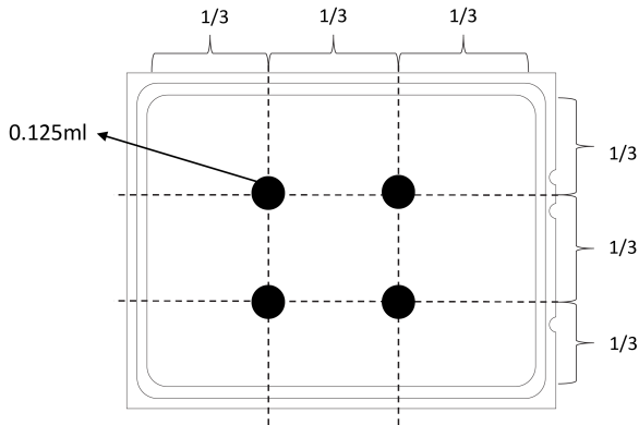
그림 135. 열전도 그리스 도포
