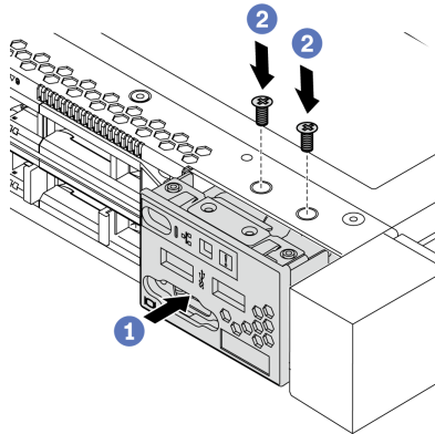
그림 46. 앞면 입/출력 어셈블리 설치
