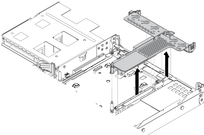
그림 112. 라이저 어셈블리 제거
