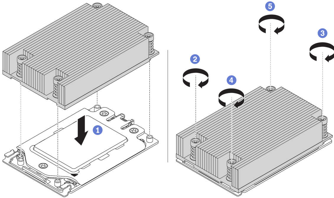
그림 134. 방열판 설치
