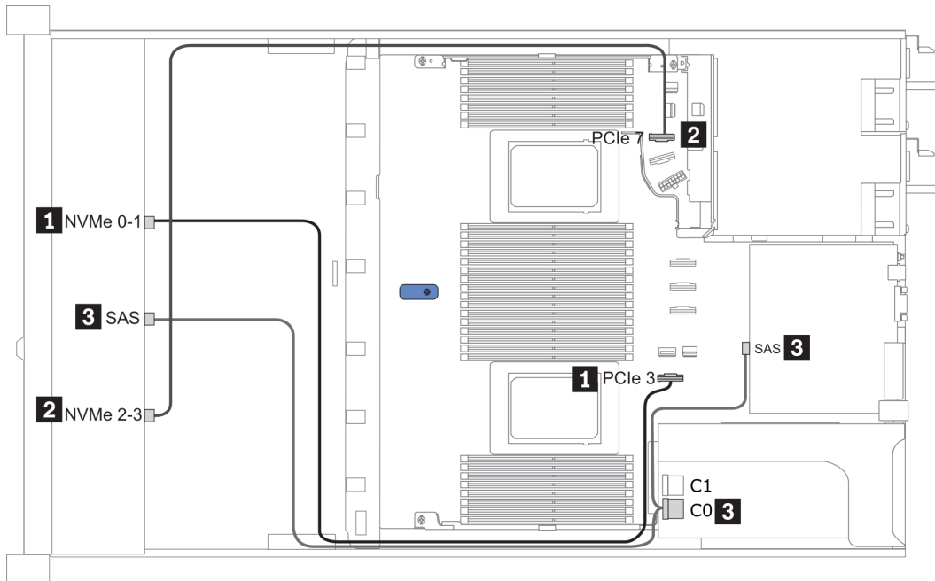
그림 37. Configuration 5
