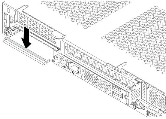
그림 93. OCP 3.0 이더넷 어댑터 레이블 설치
