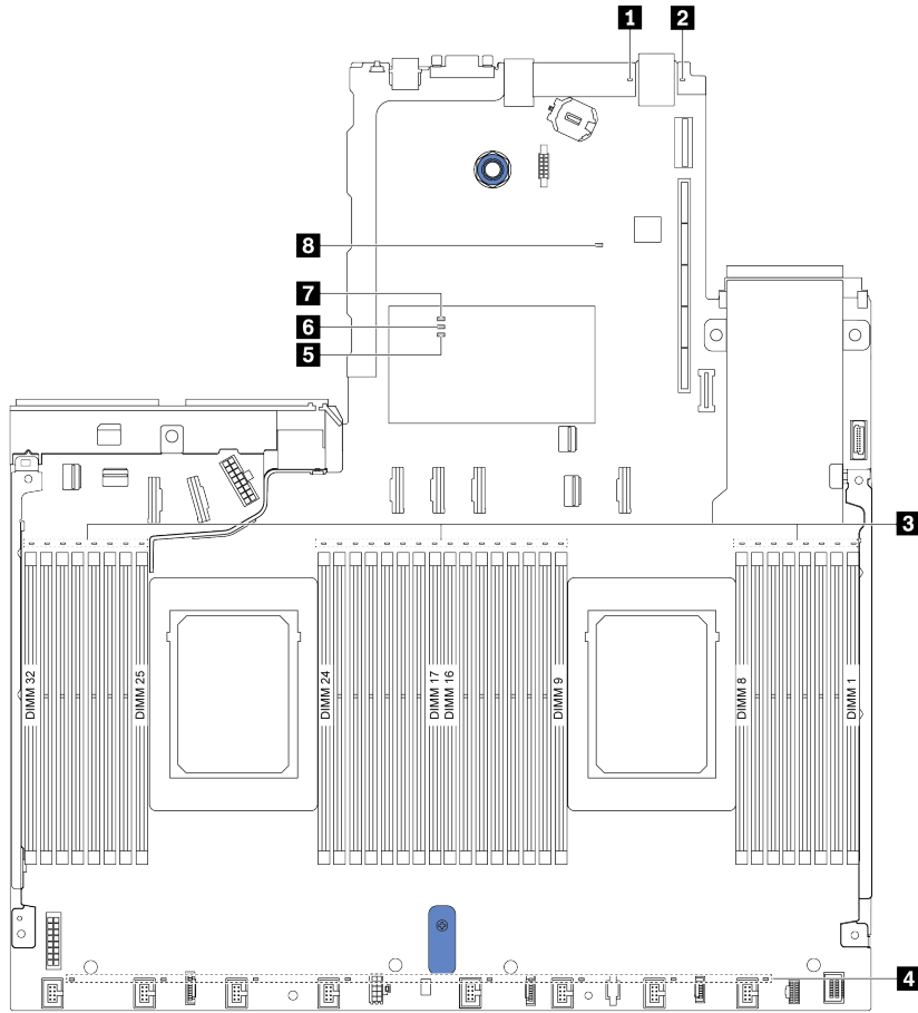
그림 10. 시스템 보드 LED
