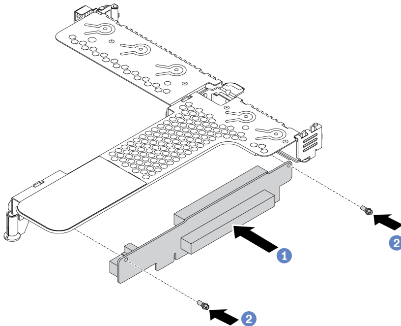
그림 115. 라이저 어셈블리 설치
