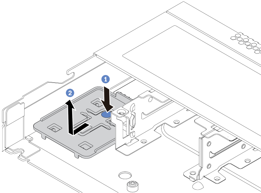
그림 105. 트레이 제거
