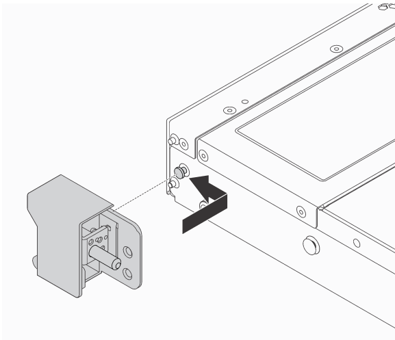
그림 100. 랙 래치 설치
