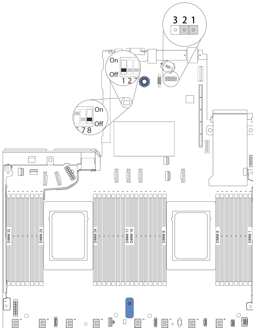
그림 11. 시스템 보드상 스위치 블록 및 점퍼 위치
