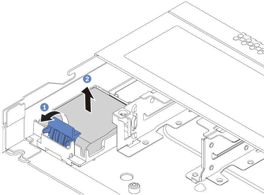
그림 103. 새시에서 RAID 슈퍼 캐패시터 모듈 제거
