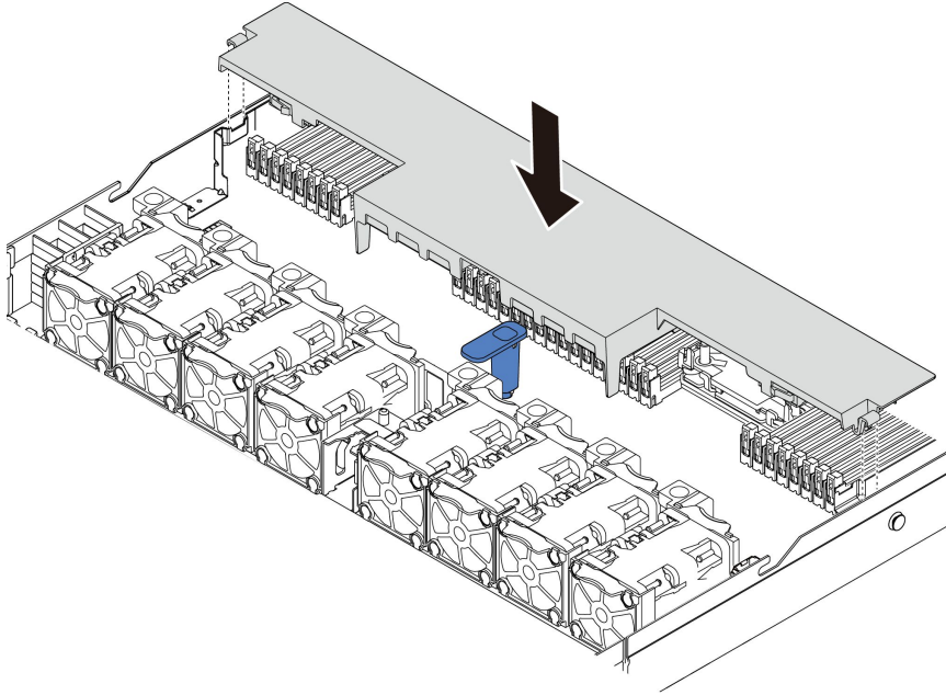
그림 41. 공기 조절 장치 설치
