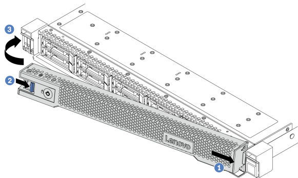
그림 122. 보안 베젤 설치
