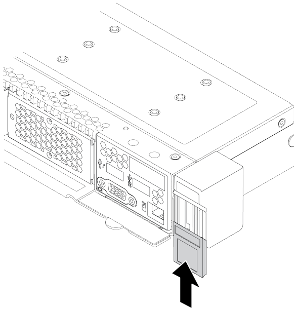
그림 102. ID 레이블판 설치
