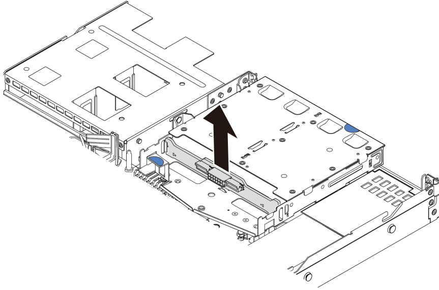
그림 61. 2.5인치 뒷면 드라이브 백플레인 제거
