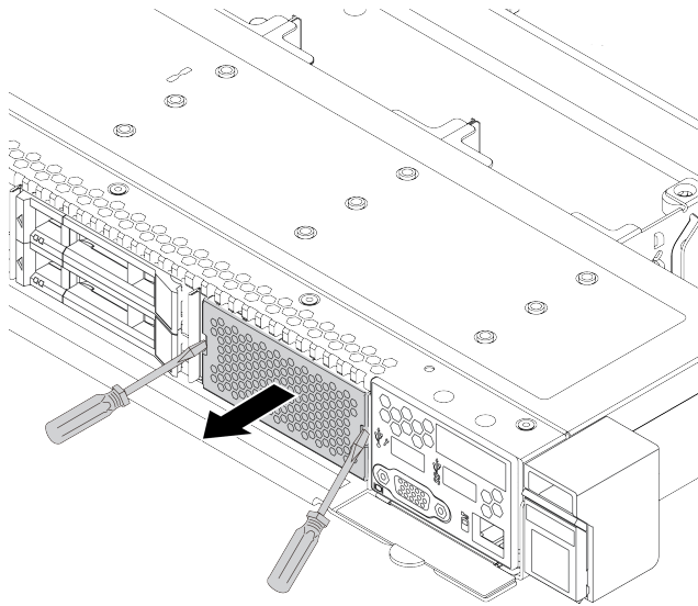
그림 49. 필터 제거
