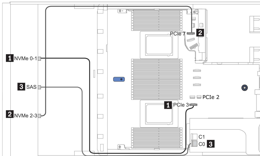
그림 36. Configuration 2
