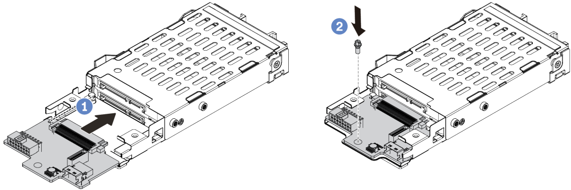
그림 66. 7mm 드라이브 백플레인 설치(하단)
