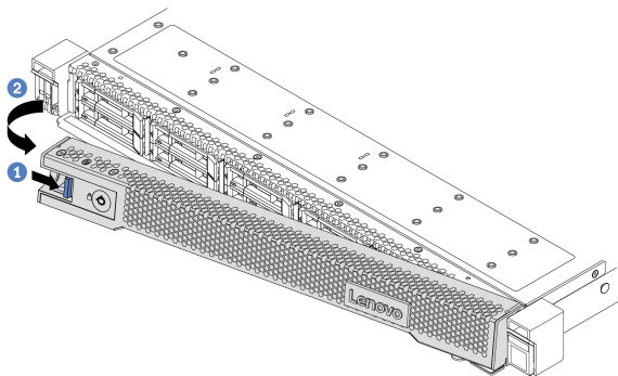
그림 120. 보안 베젤 제거
