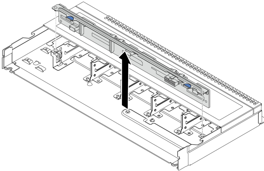
그림 56. 10개의 2.5인치 핫 스왑 드라이브용 백플레인 제거
