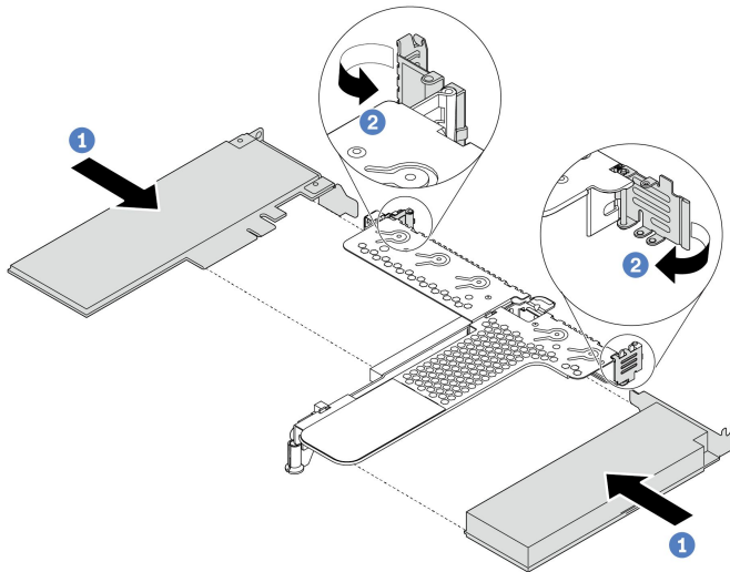
그림 96. LP-FH 라이저 어셈블리에 PCIe 어댑터 설치
