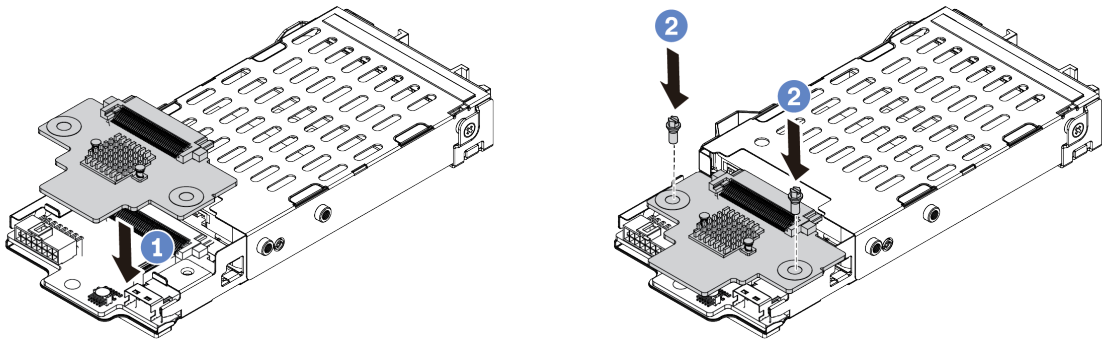
그림 67. 7mm 드라이브 백플레인 설치(상단)
