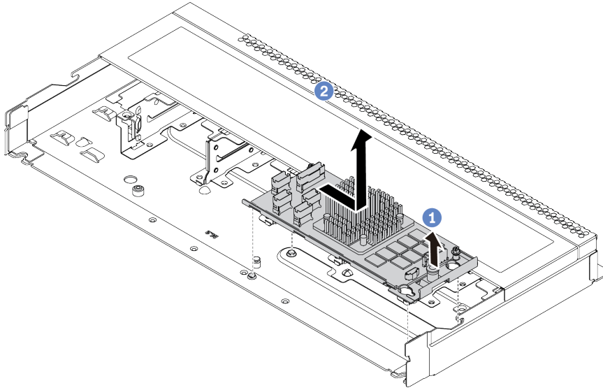
그림 79. 내부 CFF RAID/HBA 어댑터 제거
