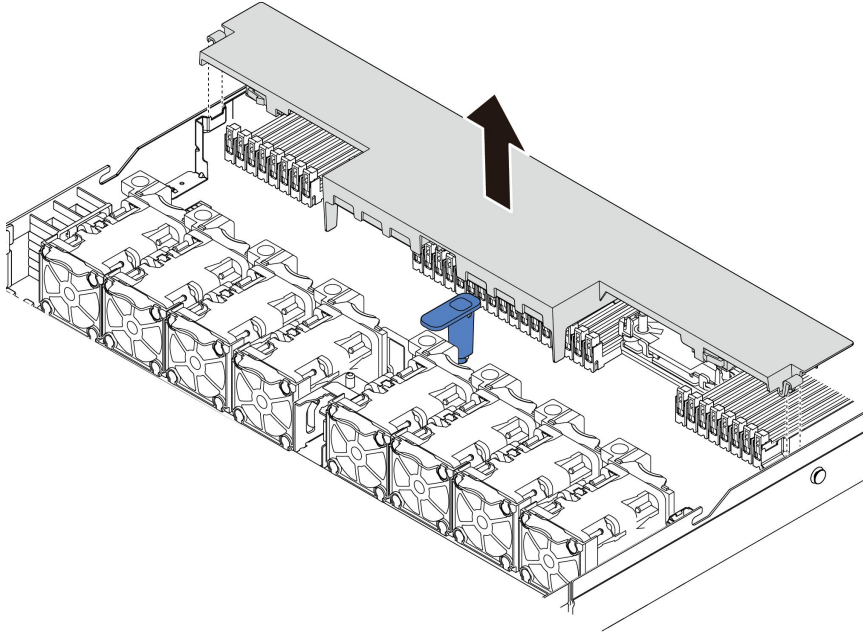
그림 40. 공기 조절 장치 제거
