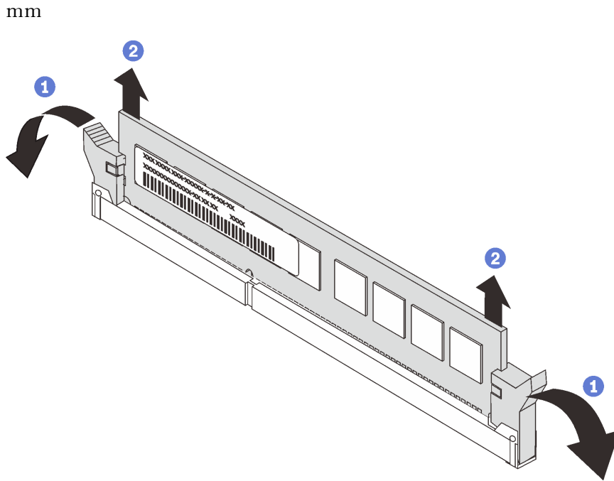
그림 83. 메모리 모듈 제거
