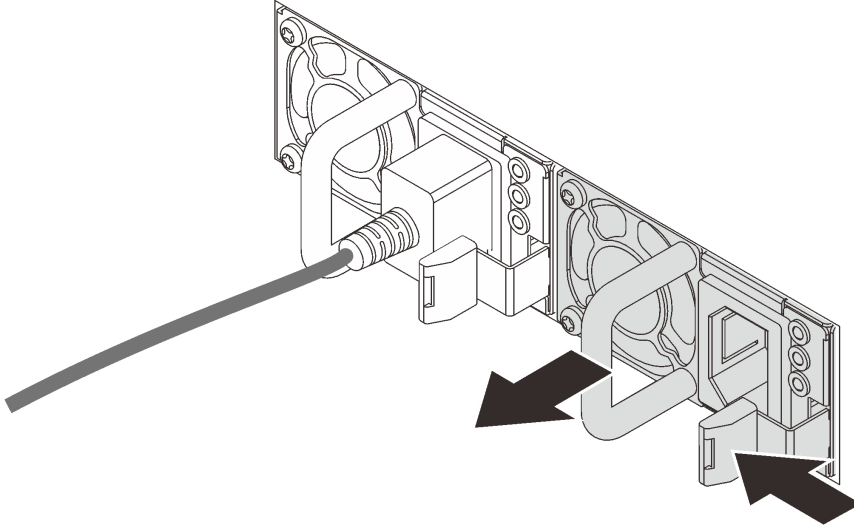
그림 74. 핫 스왑 전원 공급 장치 제거
