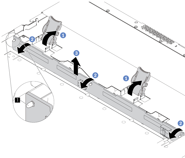
그림 58. 3.5인치 드라이브 백플레인 제거
