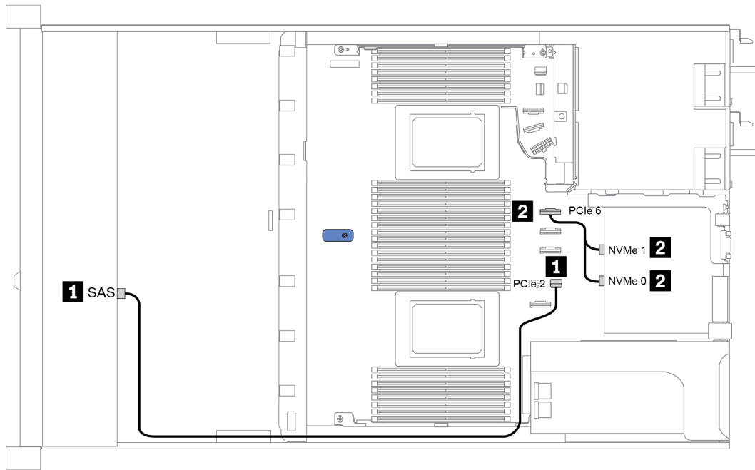
그림 35. Configuration 5
