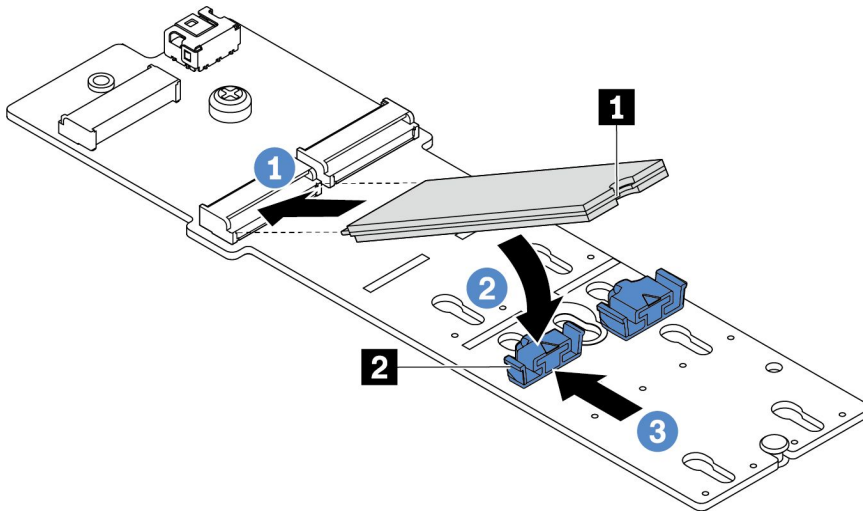
그림 91. M.2 드라이브 설치
