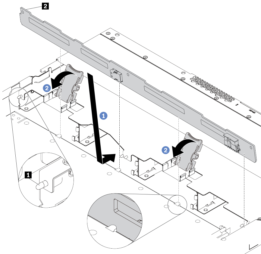
그림 59. 4개의 3.5인치 핫 스왑 드라이브용 백플레인 설치
