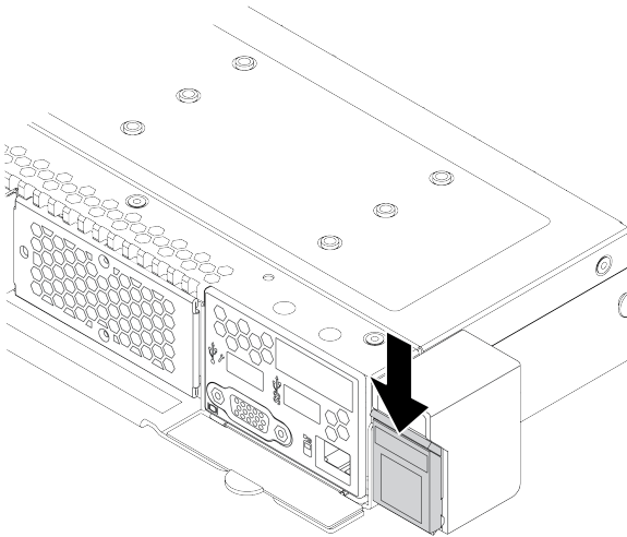
그림 97. ID 레이블판 제거
