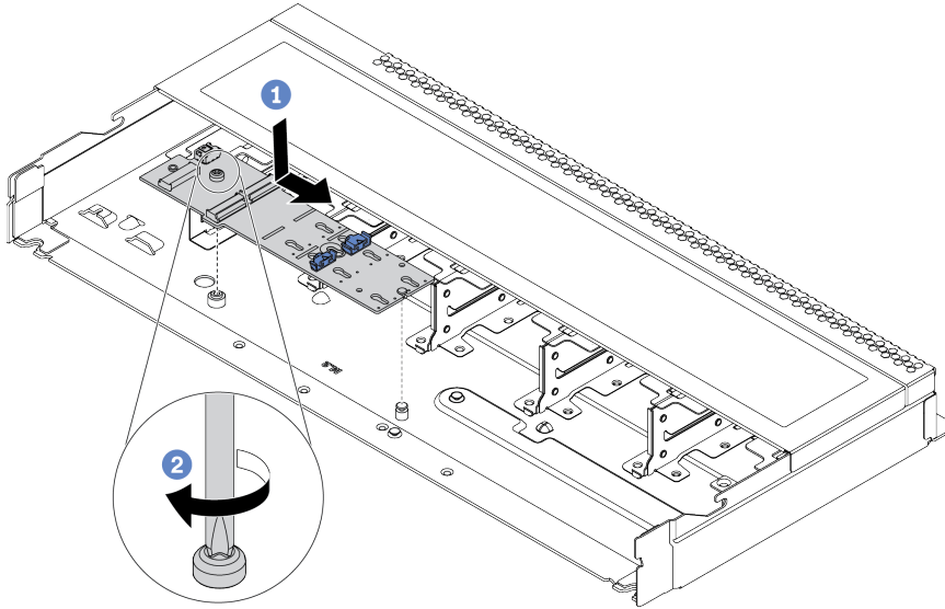
그림 90. M.2 어댑터 설치
