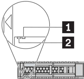
그림 4. 드라이브 LED
