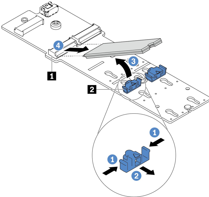
그림 85. M.2 드라이브 제거
