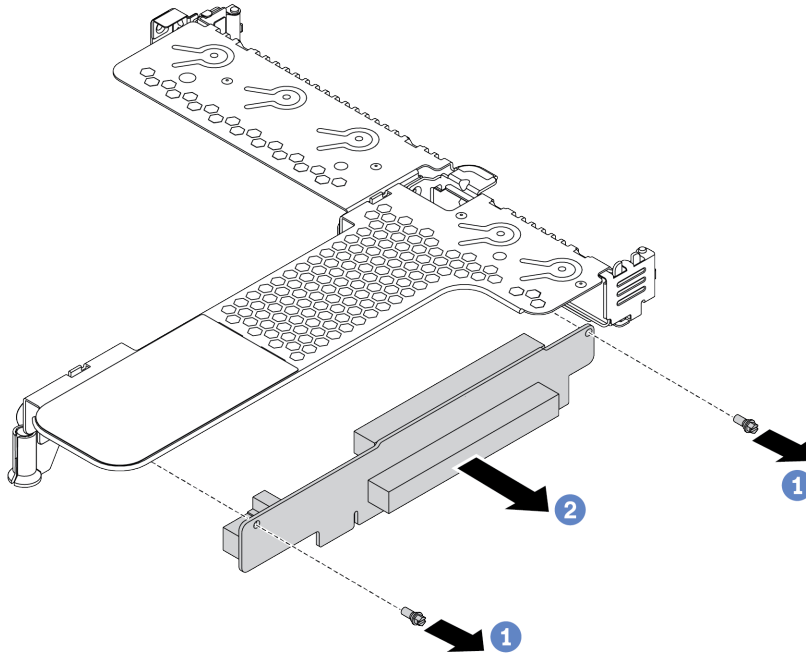
그림 113. 라이저 어셈블리 제거
