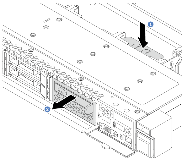
그림 47. LCD 진단 패널 어셈블리 제거
