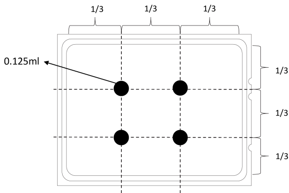
그림 133. 열전도 그리스 도포
