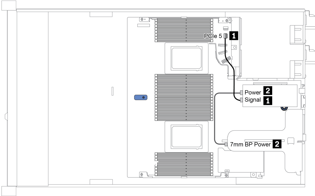
그림 15. 7mm cable routing
