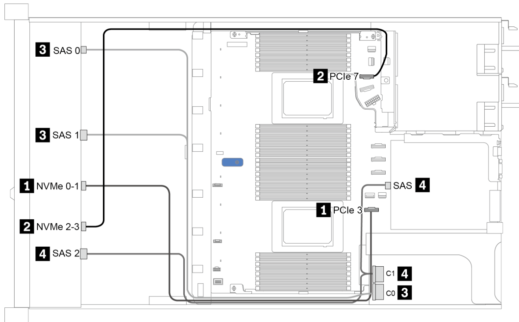
그림 21. Configuration 3
