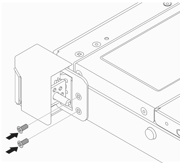
그림 101. 랙 래치 나사 설치
