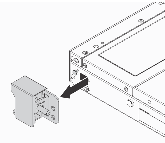
그림 99. 랙 래치 제거
