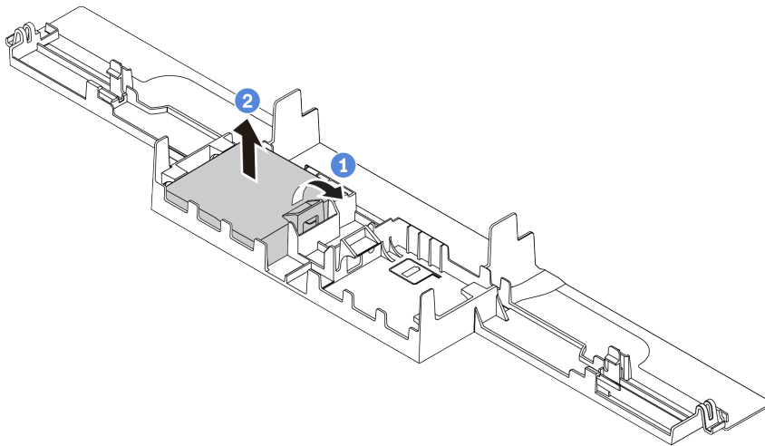
그림 108. 공기 조절 장치에서 RAID 슈퍼 캐패시터 모듈 제거
