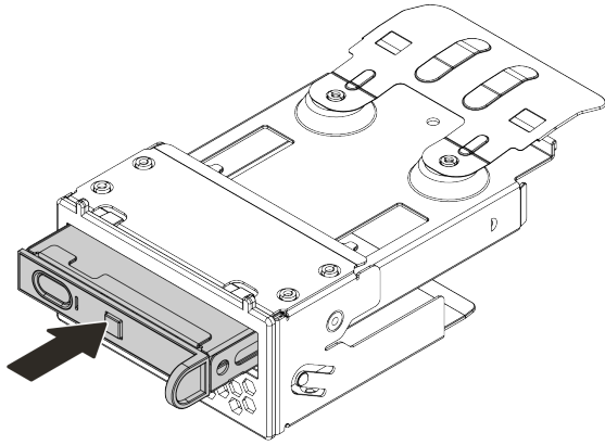
그림 50. 어셈블리에 LCD 진단 패널 설치
