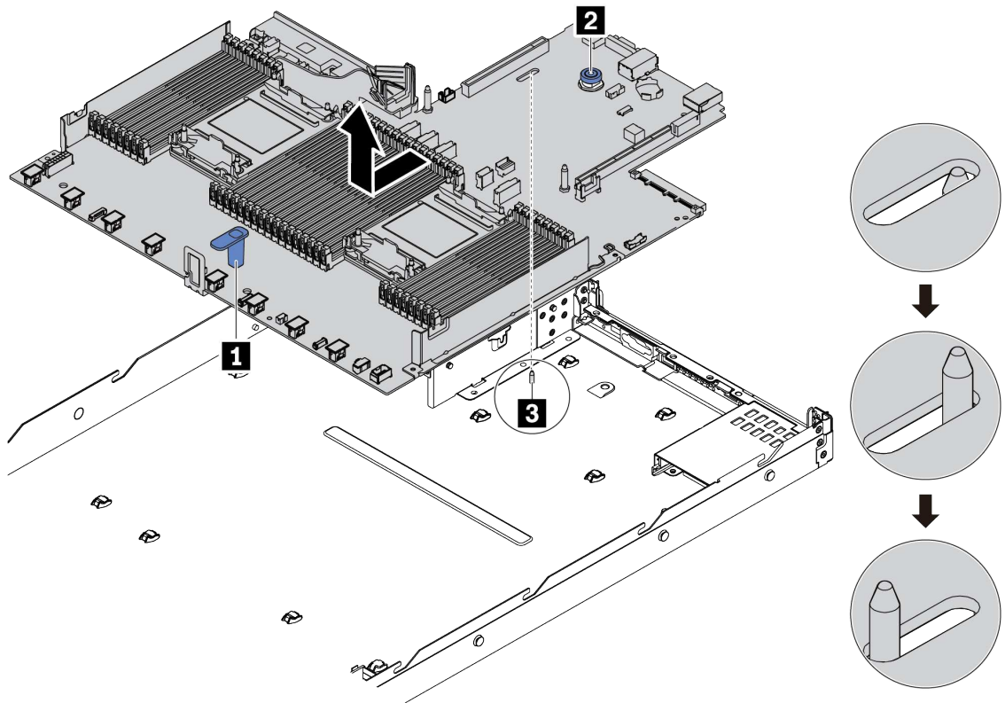
그림 138. 시스템 보드 설치
