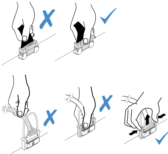
그림 44. 앞면 입/출력 어셈블리 케이블 분리
