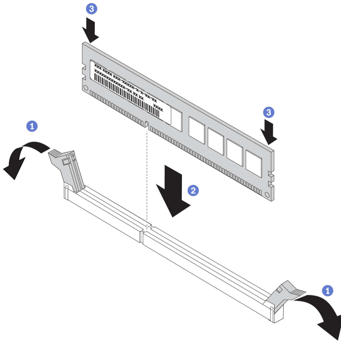
그림 84. 메모리 모듈 설치
