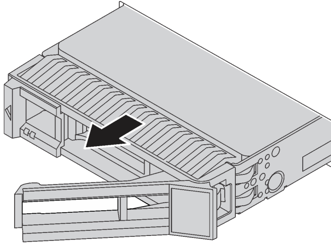
그림 53. 핫 스왑 드라이브 제거
