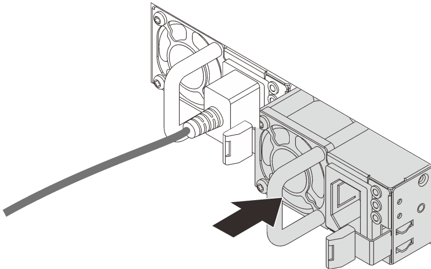
그림 77. 핫 스왑 전원 공급 장치 설치
