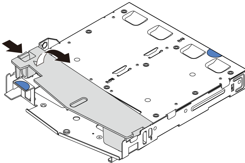
그림 69. 공기 조절 장치 제거
