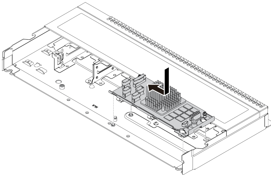
그림 80. 내부 CFF RAID/HBA 어댑터 설치
