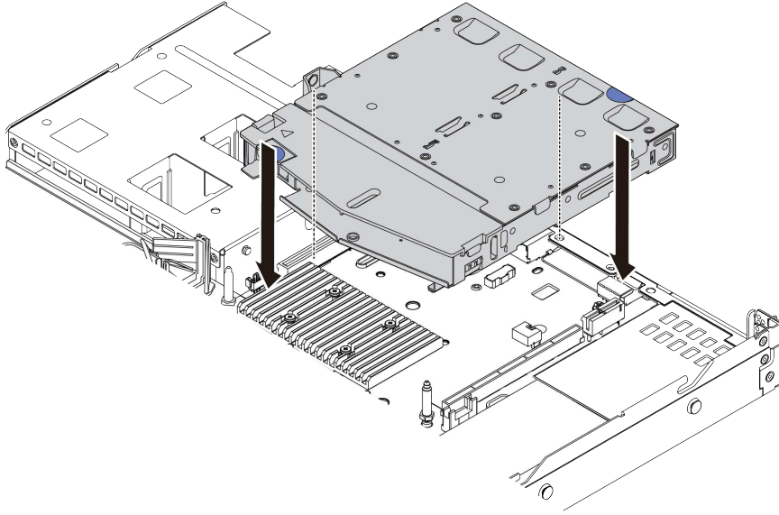
그림 72. 핫 스왑 뒷면 드라이브 케이지 설치
