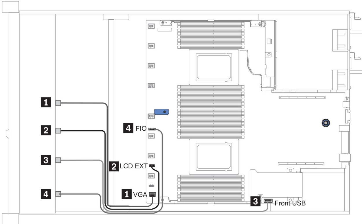
그림 12. FIO cable routing
