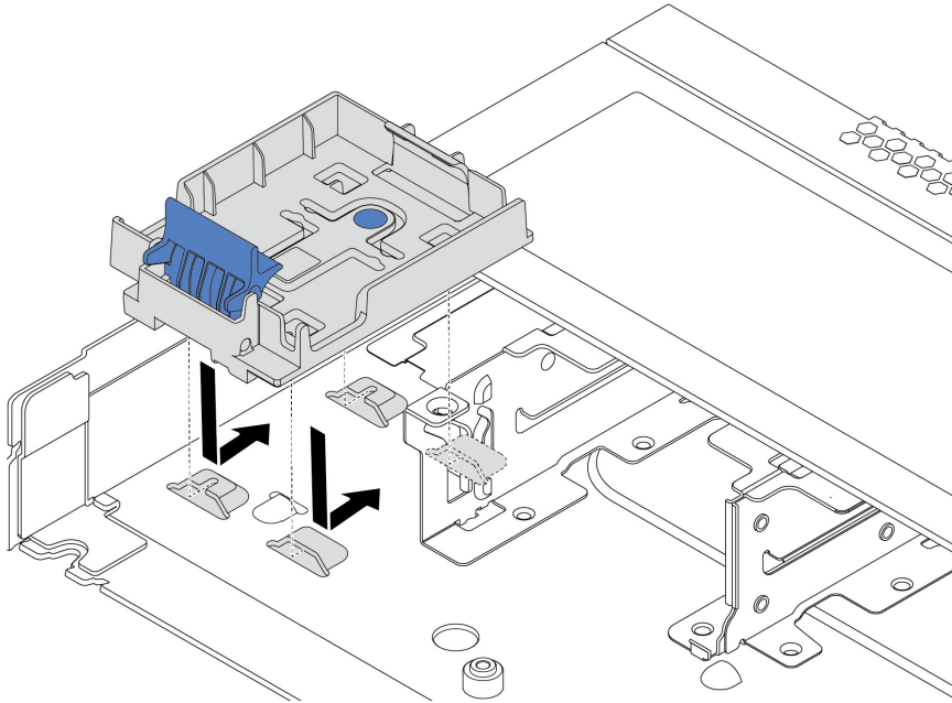
그림 106. RAID 슈퍼 커패시터 모듈 홀더 설치
