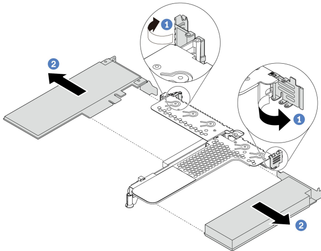
그림 95. LP-FH 라이저 어셈블리에서 PCIe 어댑터 제거
