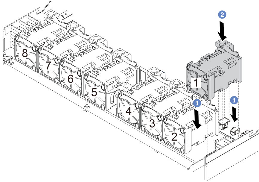
그림 118. 시스템 팬 설치
