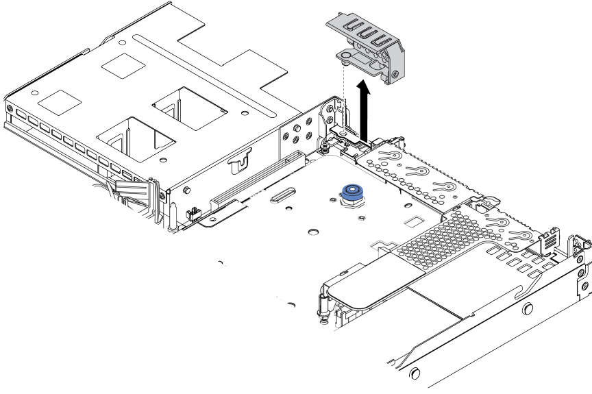
그림 114. 뒷면 벽 브래킷 제거
