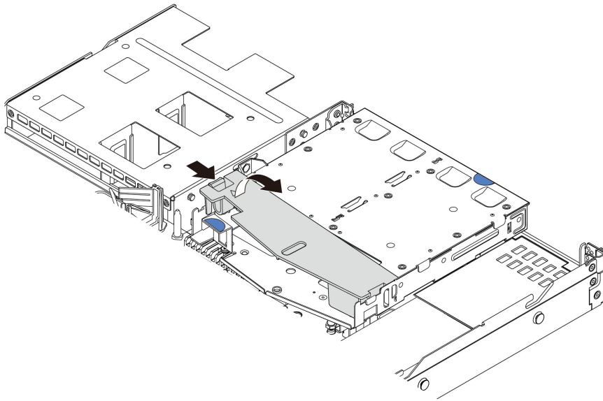
그림 60. 공기 조절 장치 제거
