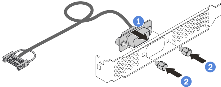
그림 126. 직렬 포트 모듈 설치
