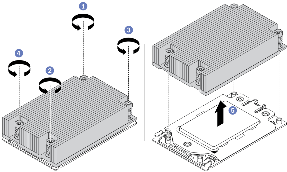
그림 129. 방열판 제거
