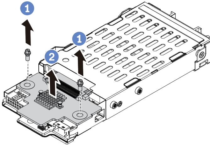
그림 64. 7mm 드라이브 백플레인 제거(상단)
