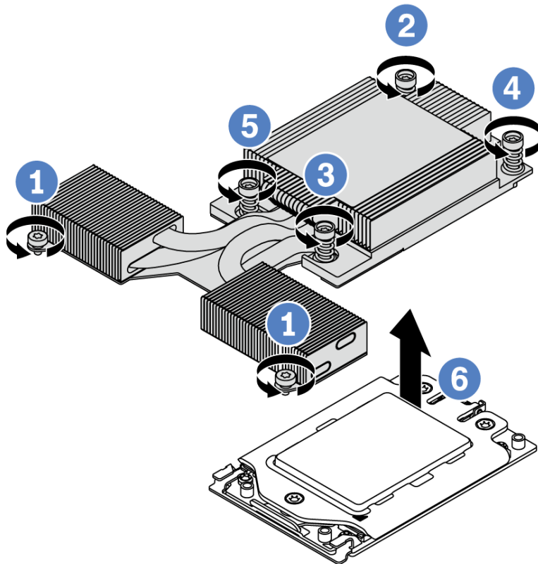
그림 130. 방열판 제거
