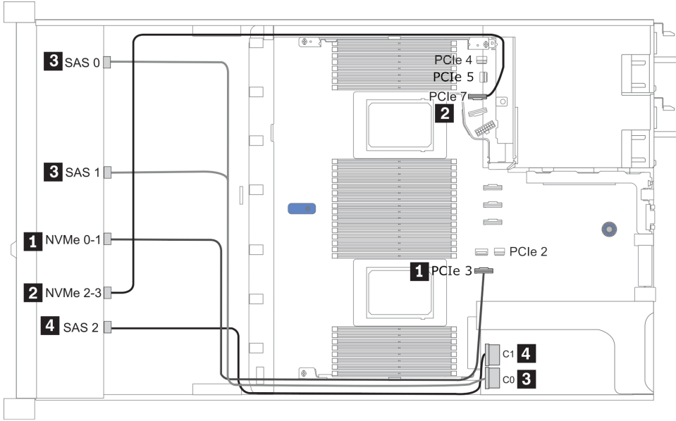
그림 28. Configuration 2 (2 CPU installed)
