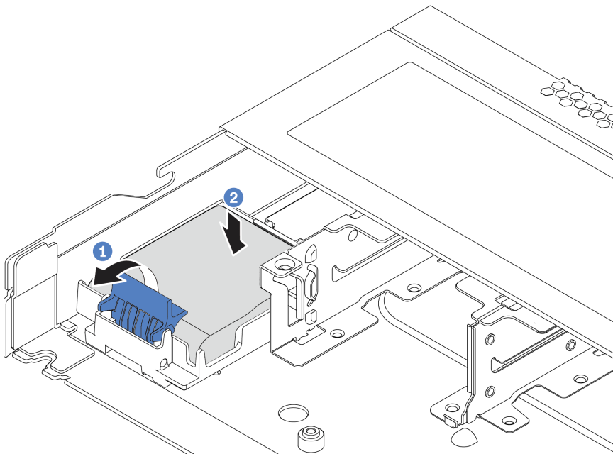
그림 107. 새시에 RAID 슈퍼 커패시터 모듈 설치
