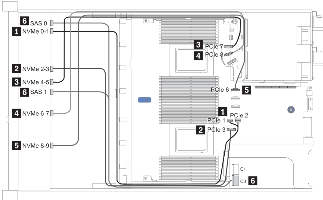
그림 27. Configuration 1
