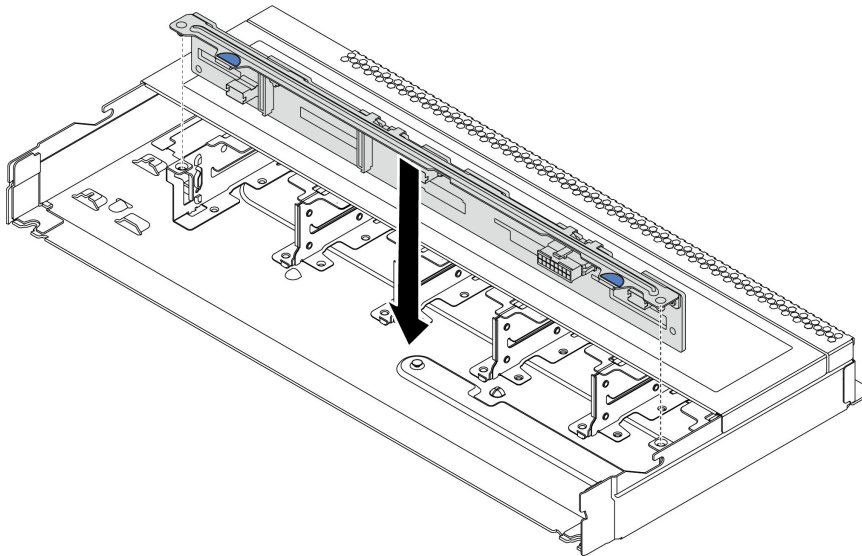
그림 57. 10개의 2.5인치 핫 스왑 드라이브용 백플레인 설치
