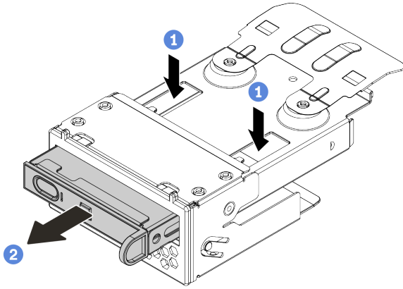
그림 48. LCD 진단 패널 제거
