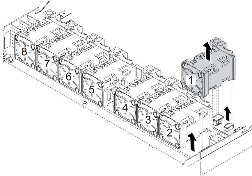
그림 117. 시스템 팬 제거
