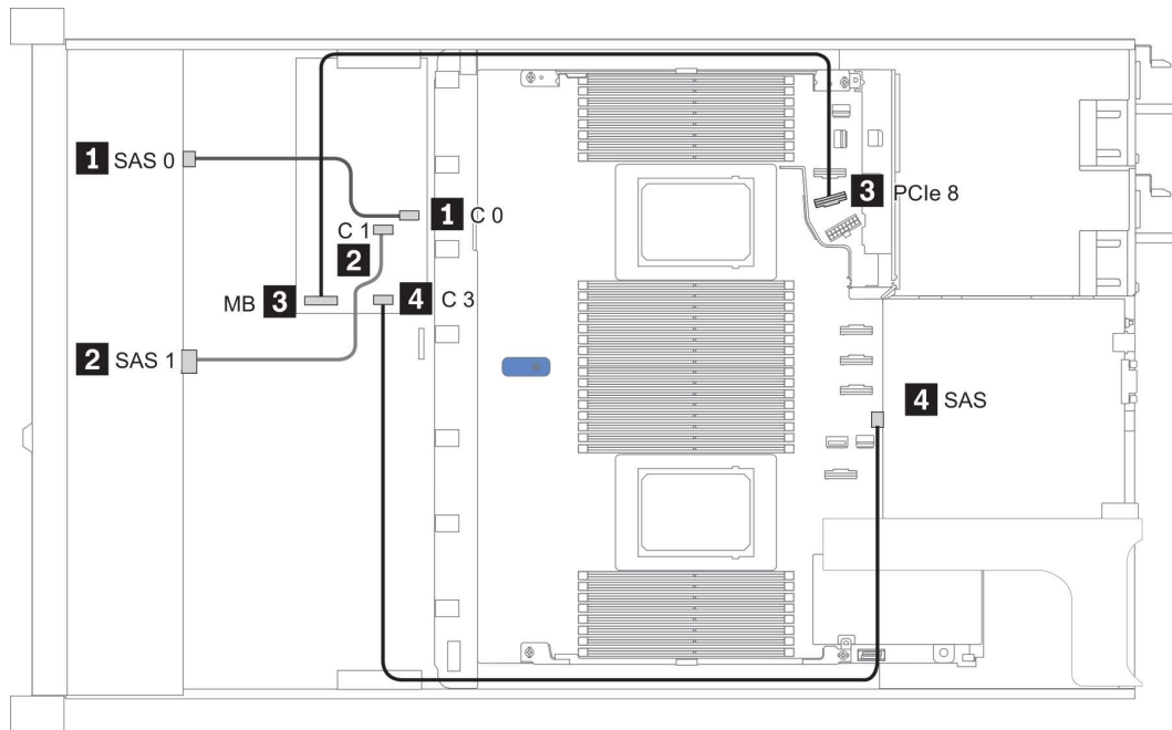
그림 19. Configuration 6
