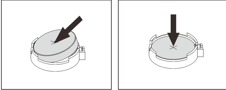
그림 43. CMOS 배터리 설치
