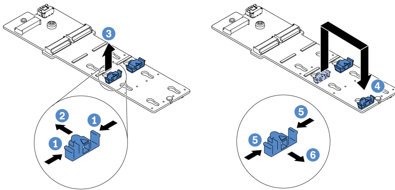
그림 88. M.2 고정장치 조정
