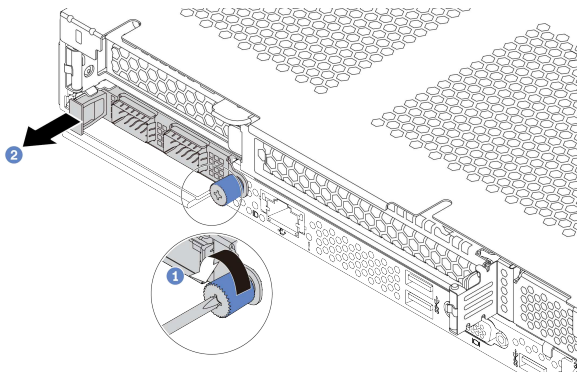
그림 92. OCP 3.0 이더넷 어댑터 제거
