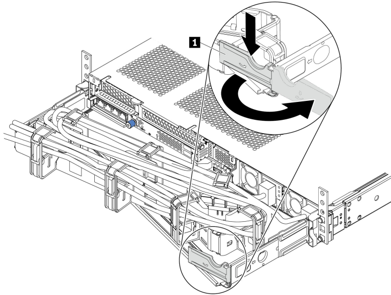
그림 73. CMA 조정
