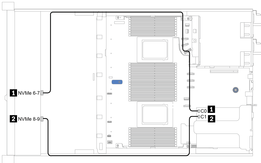
그림 39. Configuration 1
