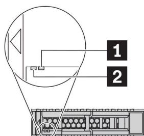
圖例 6. 硬碟 LED
