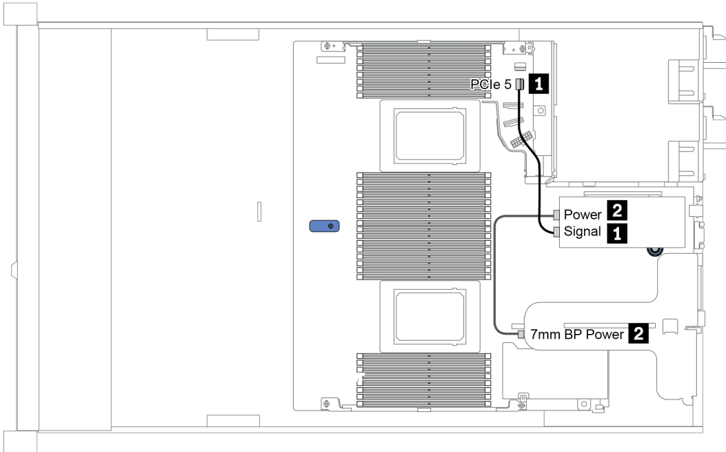
圖例 13. 7mm cable routing
