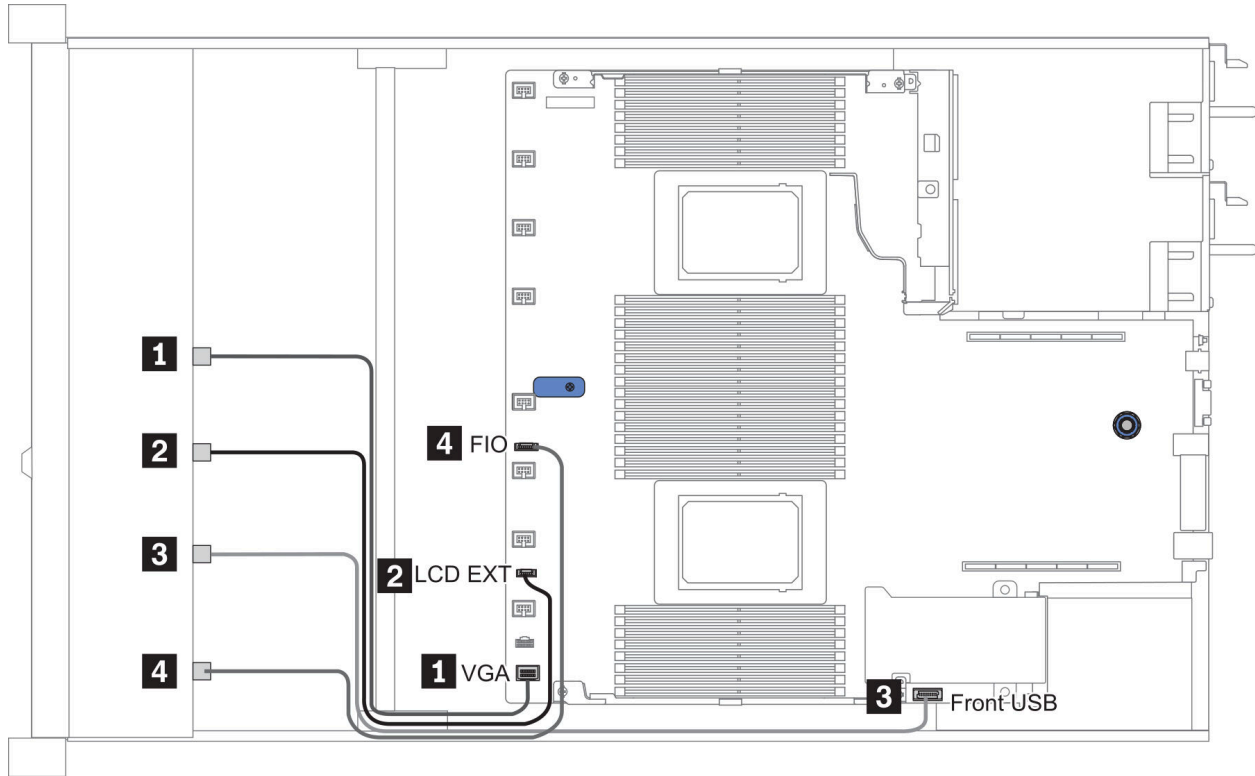
圖例 10. FIO cable routing
