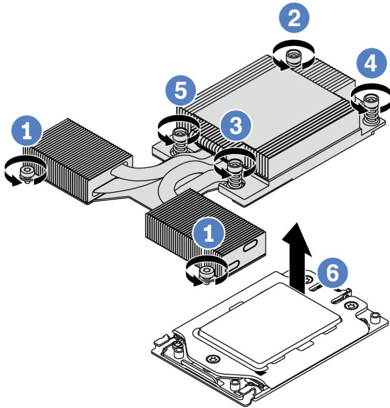
圖例 47. 效能散熱槽安裝
