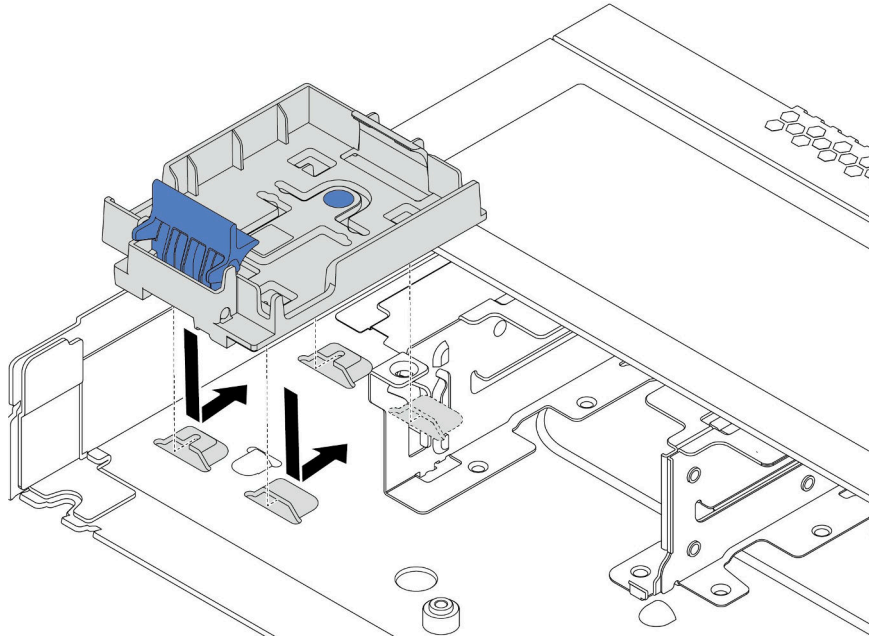
圖例 76. 安裝 RAID 超級電容器模組匣
