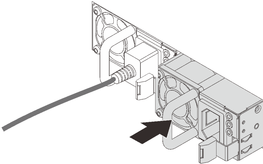
圖例 86. 安裝熱抽換電源供應器
