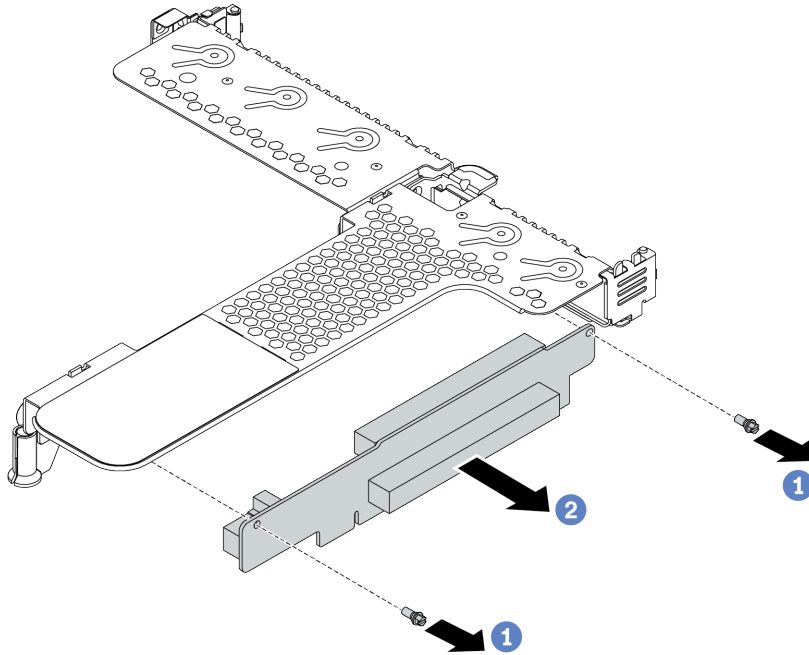
圖例 43. 移除擴充卡
