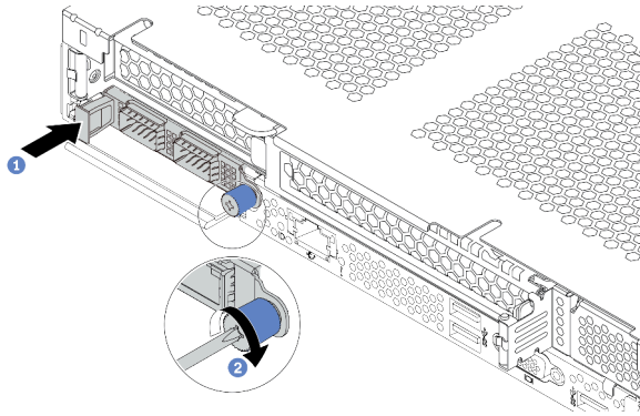
圖例 79. OCP 3.0 乙太網路配接卡安裝
