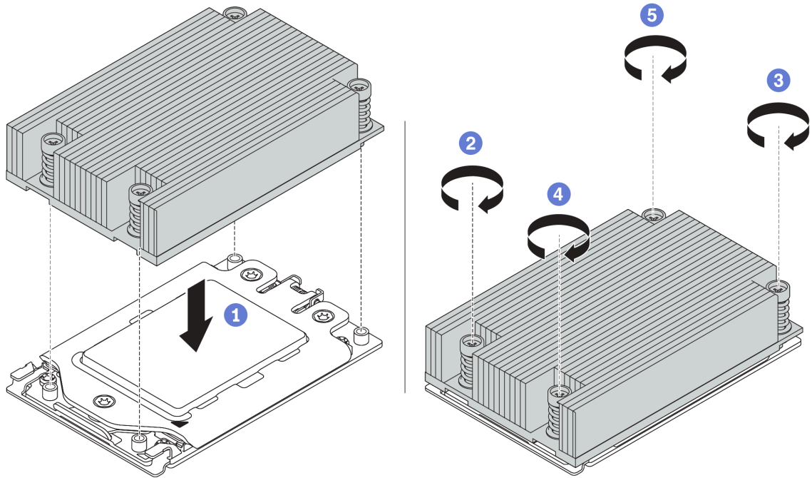
圖例 46. 標準散熱槽安裝
