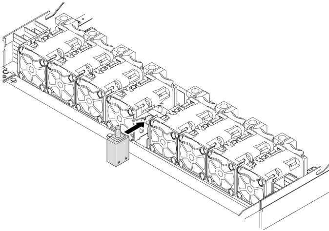
圖例 81. 入侵開關安裝
