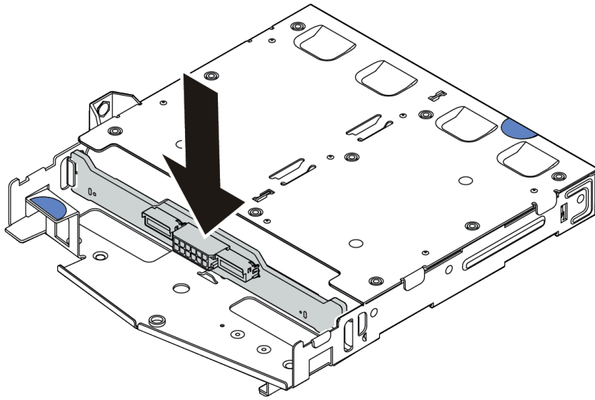
圖例 64. 安裝後方背板
