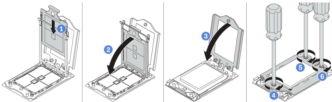
圖例 45. 安裝處理器
