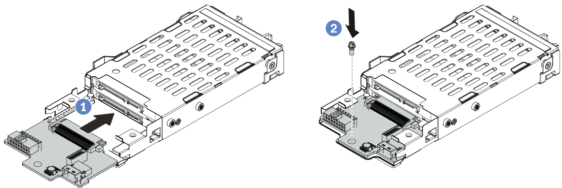
圖例 51. 7 公釐硬碟背板安裝（底部）
