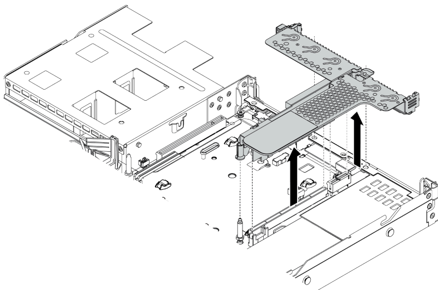
圖例 42. 卸下擴充卡組件
