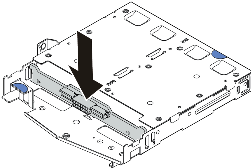
圖例 54. 安裝後方背板
