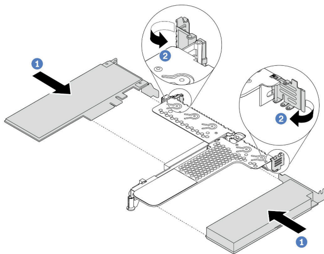
圖例 67. 將 PCIe 配接卡安裝在 LPFH 擴充卡組件中
