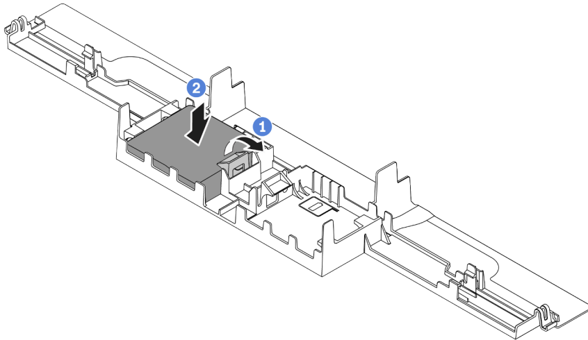
圖例 74. 在空氣擋板上安裝 RAID 超級電容器模組
