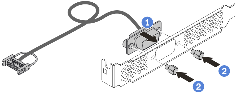
圖例 70. 序列埠模組安裝
