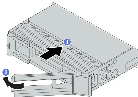
圖例 62. 熱抽換硬碟安裝
