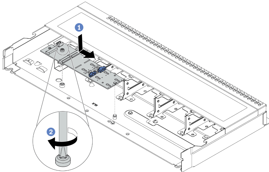
圖例 57. M.2 配接卡安裝
