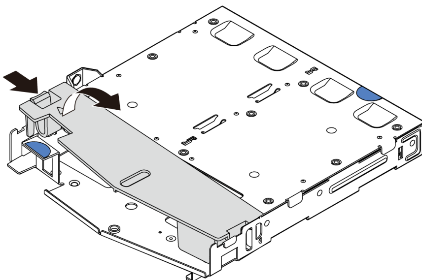
圖例 63. 卸下空氣擋板
