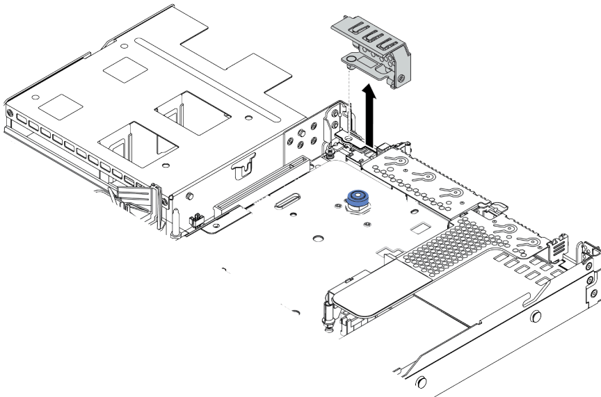
圖例 44. 卸下後壁托架
