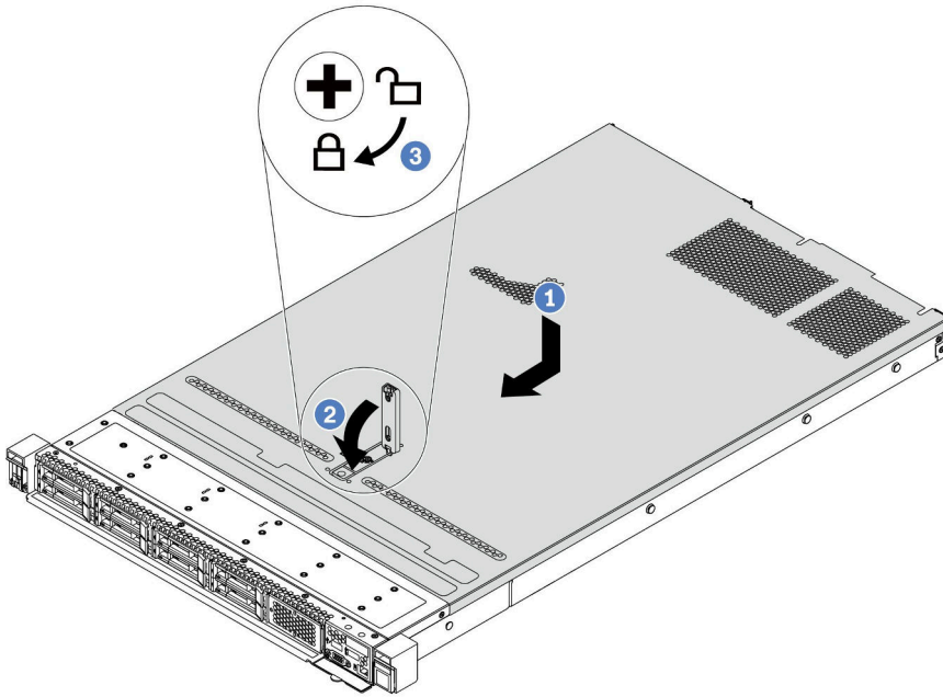
圖例 83. 安裝上蓋
