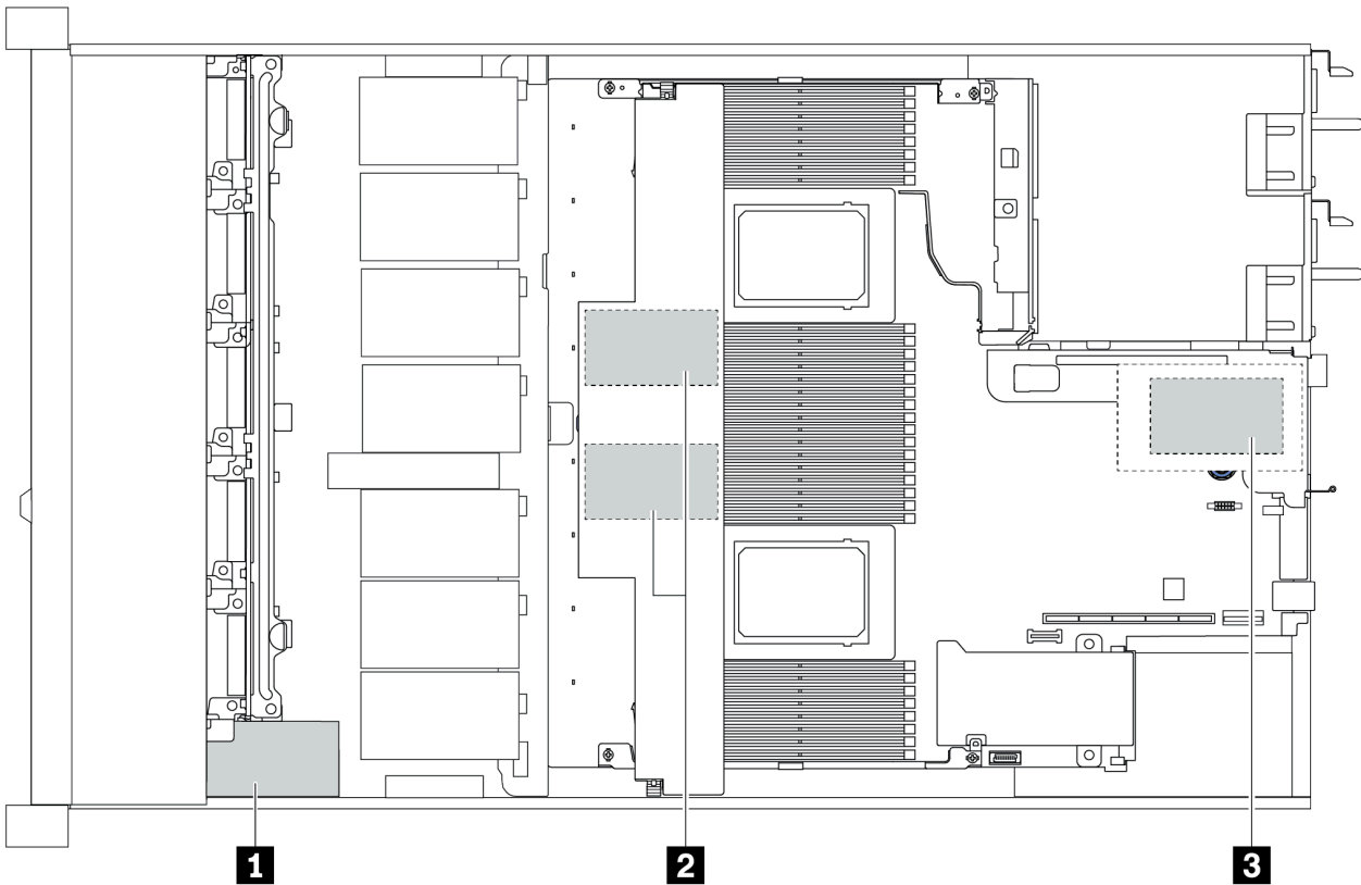
圖例 72. RAID 超級電容器模組位置
