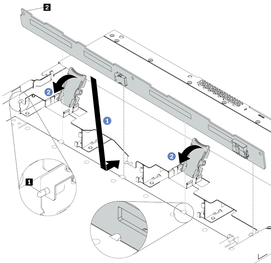
圖例 50. 安裝四個 3.5 吋熱抽換硬碟的背板
