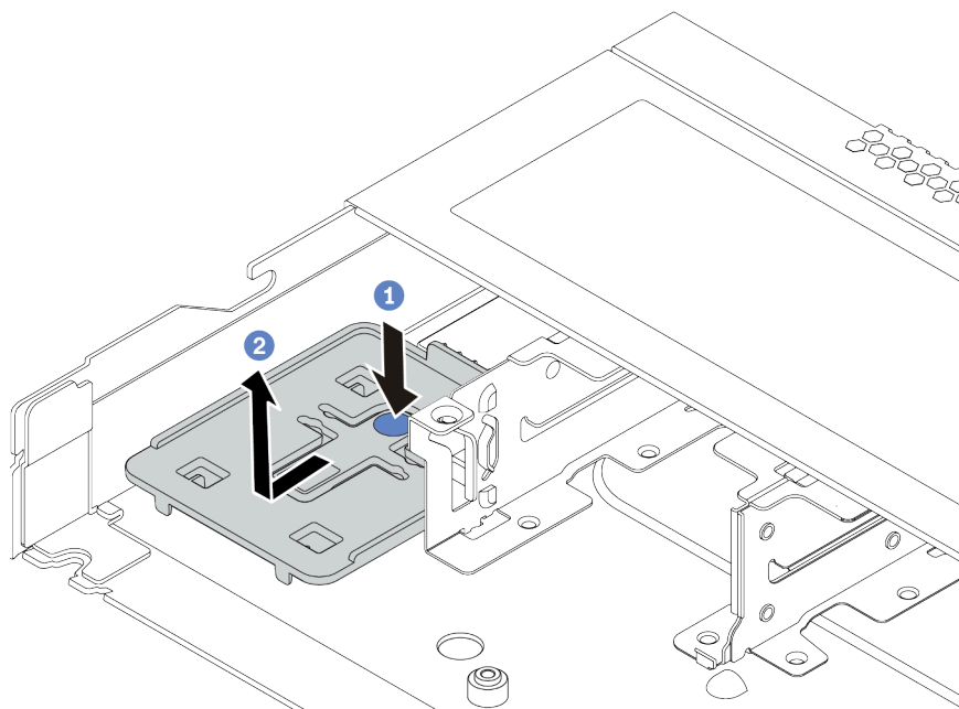
圖例 75. 卸下托盤
