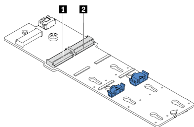
圖例 56. M.2 硬碟插槽
