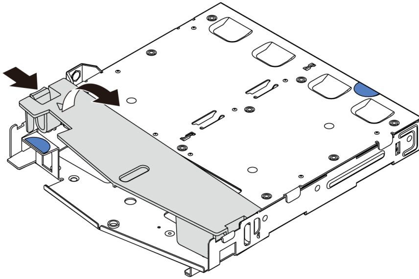
圖例 53. 卸下空氣擋板
