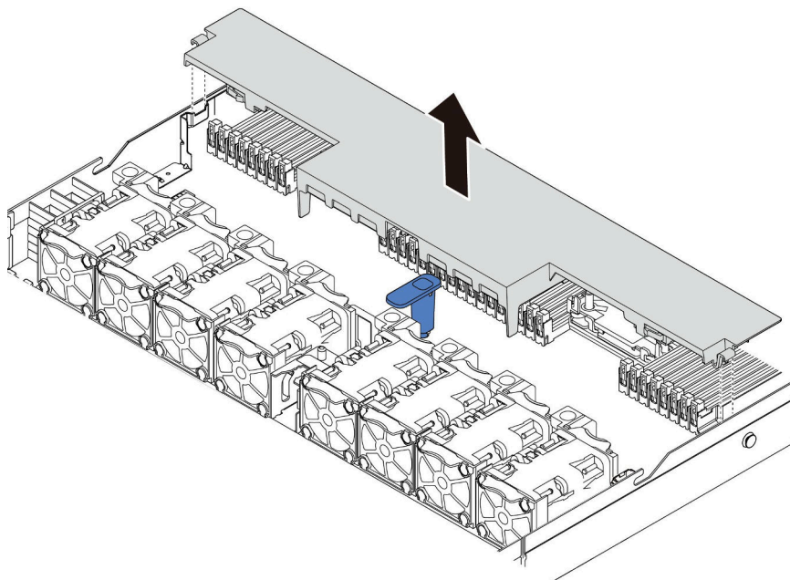
圖例 41. 卸下空氣擋板
