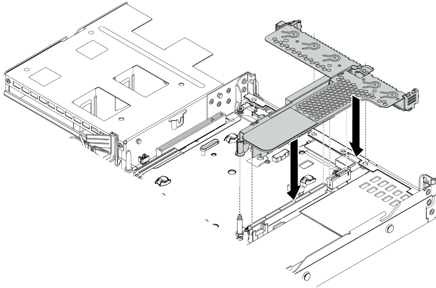
圖例 68. 安裝擴充卡組件
