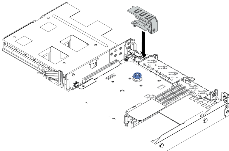
圖例 69. 後壁托架安裝
