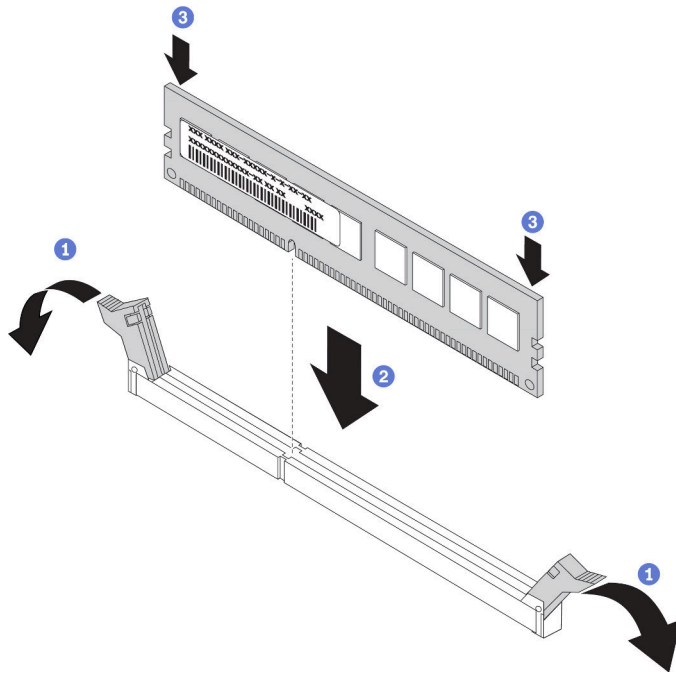
圖例 48. 安裝記憶體模組
