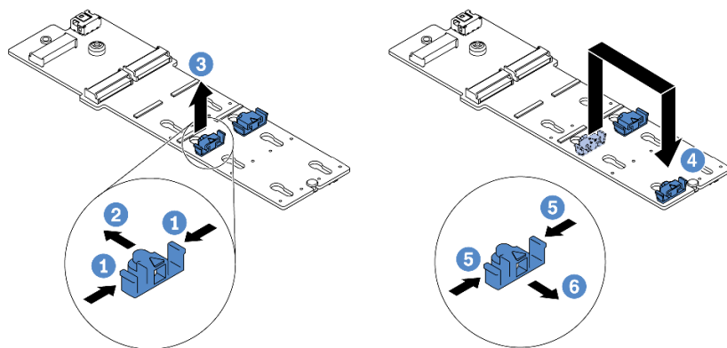
圖例 60. 調整 M.2 固定器
