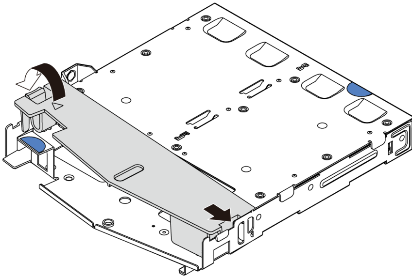
圖例 65. 安裝空氣擋板
