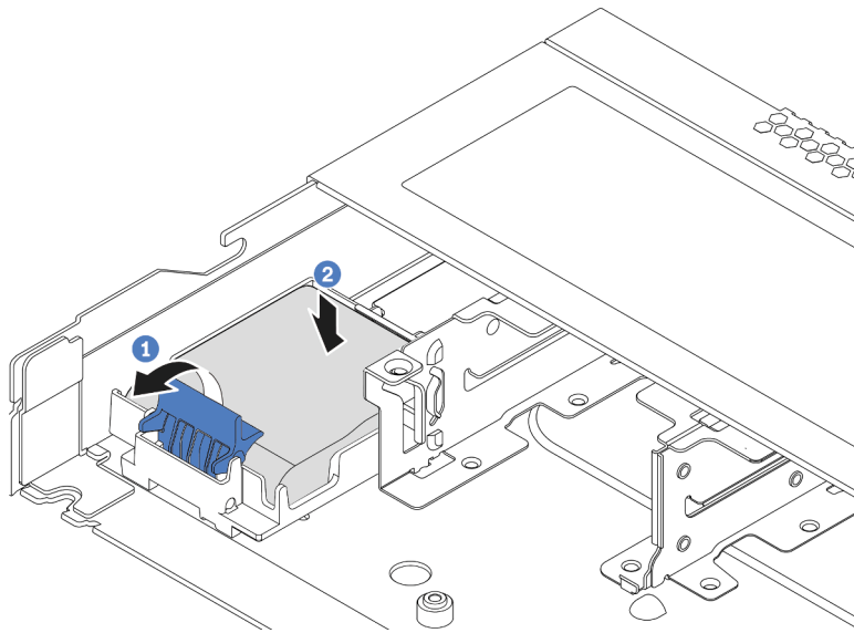
圖例 77. 安裝機箱上的 RAID 超級電容器模組
