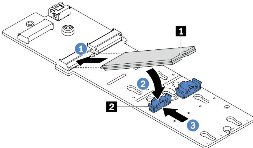
圖例 58. M.2 硬碟安裝
