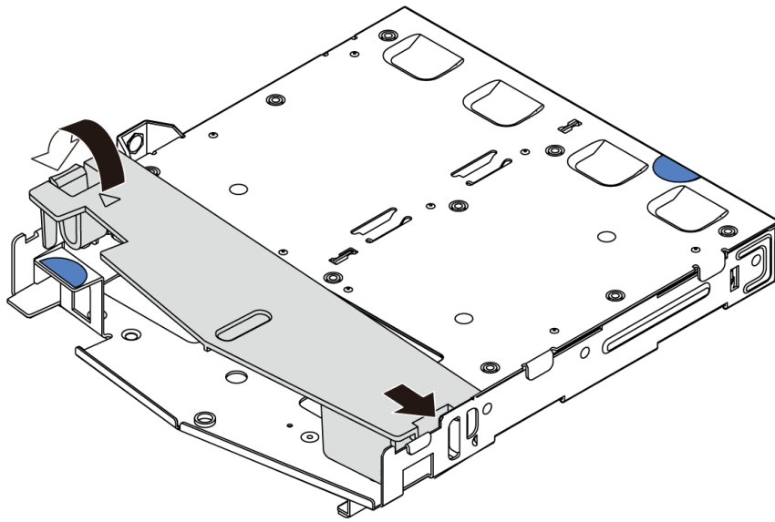
圖例 55. 安裝空氣擋板
