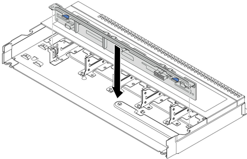
圖例 49. 安裝十個 2.5 吋熱抽換硬碟的背板
