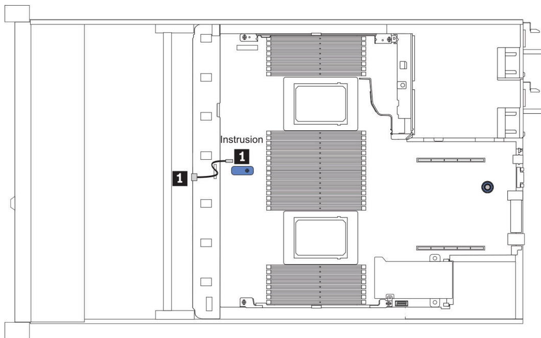
圖例 11. 入侵開關纜線佈線
