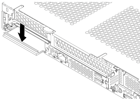
圖例 78. OCP 3.0 乙太網路配接卡標籤安裝
