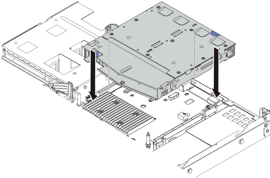
圖例 66. 安裝背面熱抽換硬碟框架
