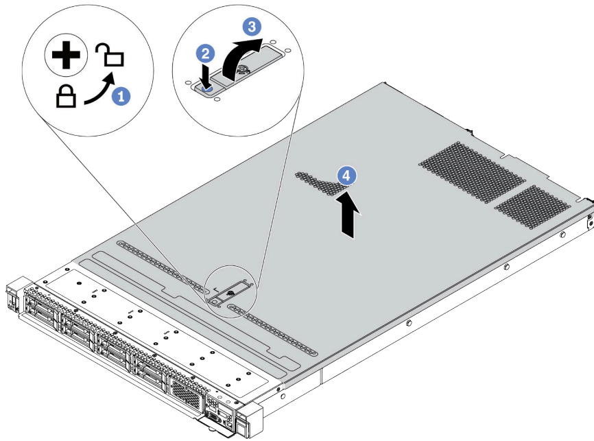
圖例 40. 卸下上蓋
