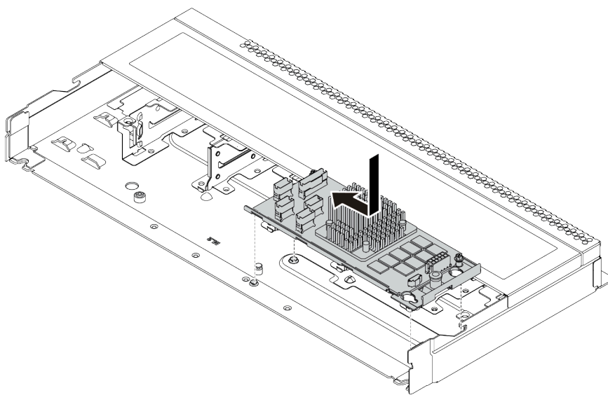
圖例 71. 安裝內部 RAID 配接卡
