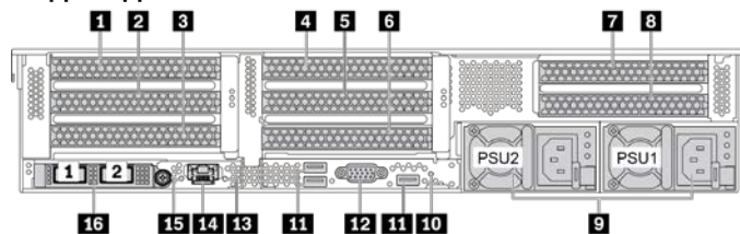
Рисунок 8. Вид сзади с восемью гнездами PCIe
