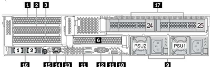
Рисунок 11. Вид сзади с четырьмя гнездами PCIe и двумя отсеками для 3,5-дюймовых дисков
