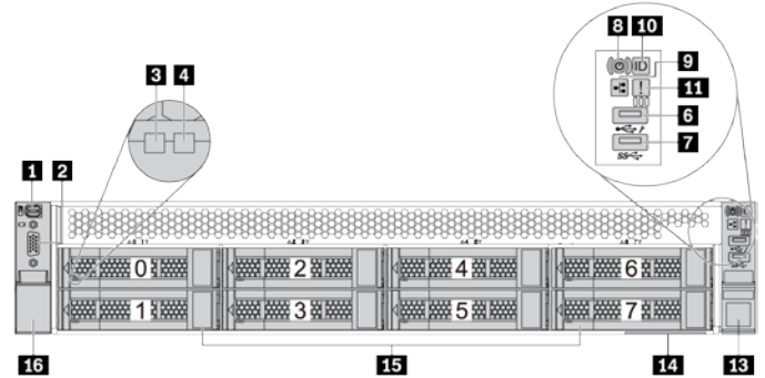
Рисунок 6. Вид спереди с 8 отсеками для 3,5-дюймовых дисков
