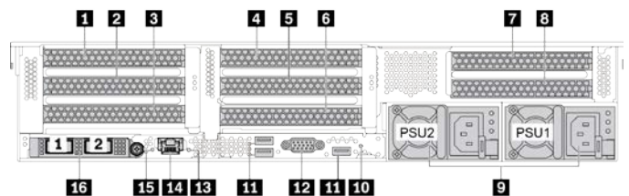
Рисунок 8. Вид сзади с восемью гнездами PCIe
