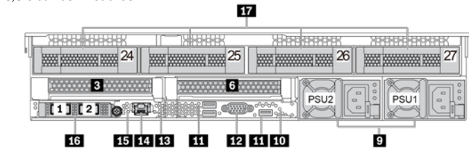
Рисунок 12. Вид сзади с двумя гнездами PCIe и четырьмя отсеками для 3,5-дюймовых дисков
