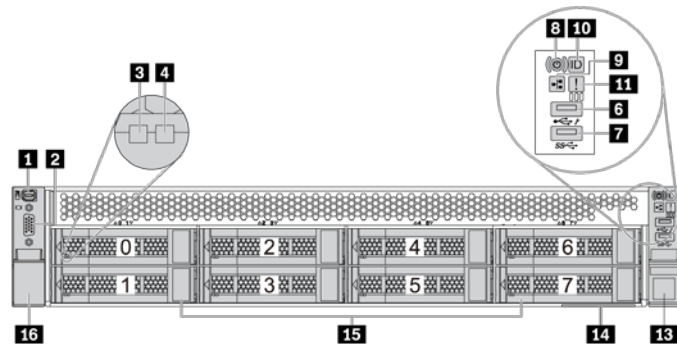
Рисунок 6. Вид спереди с 8 отсеками для 3,5-дюймовых дисков
