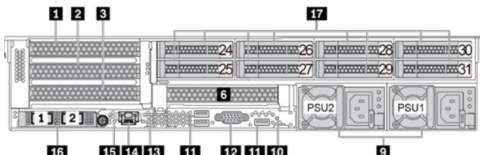
Рисунок 10. Вид сзади с четырьмя гнездами PCIe и восемью отсеками для 2,5-дюймовых дисков
