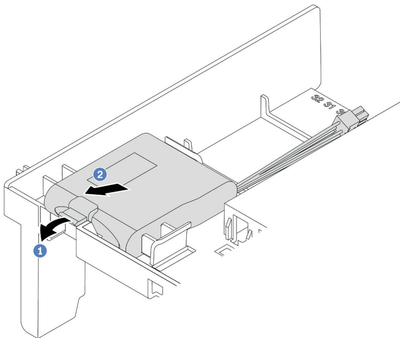
图 300. 卸下 RAID 快速充电模块
