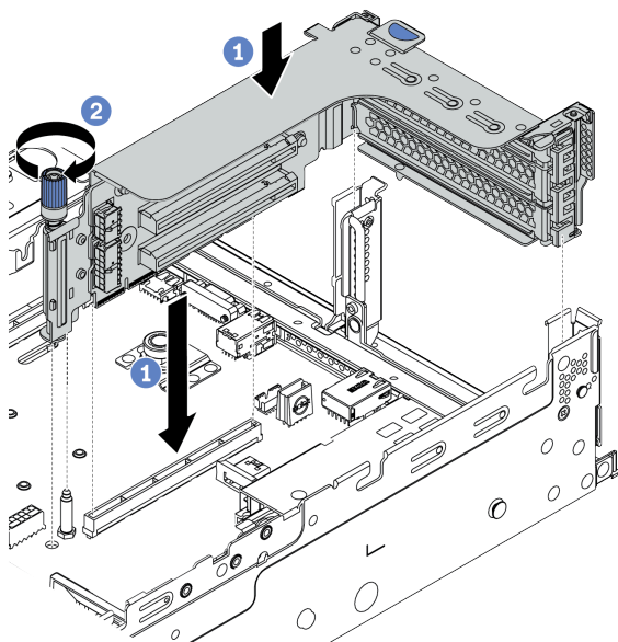
图 267. 安装转接卡组合件
