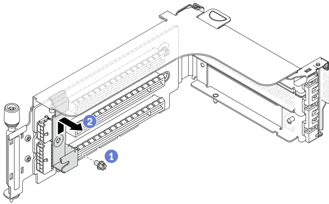
图 330. 卸下 7 毫米硬盘仓固定夹
