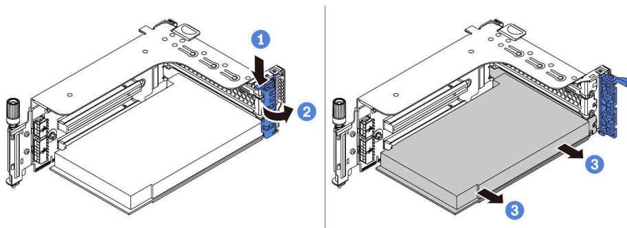
图 263. 卸下 PCIe 适配器
