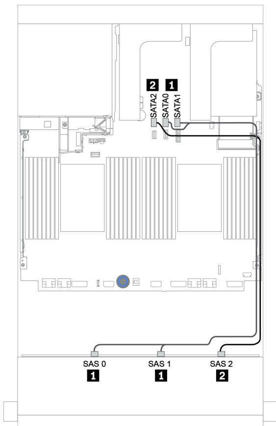
图 149. 配备板载接口的 12 x 3.5 英寸 SAS/SATA 配置的线缆布放
