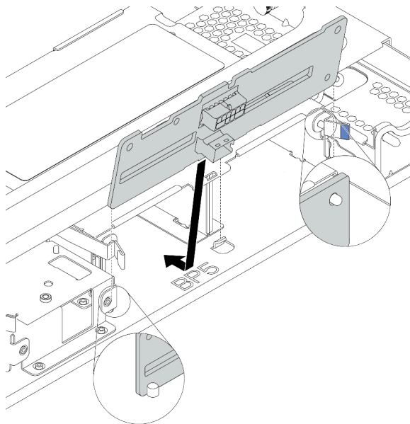
图 254. 安装 2.5 英寸中间硬盘背板
