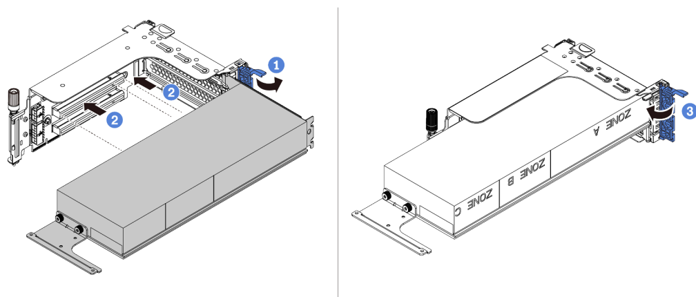
图 221. 安装 GPU 适配器
