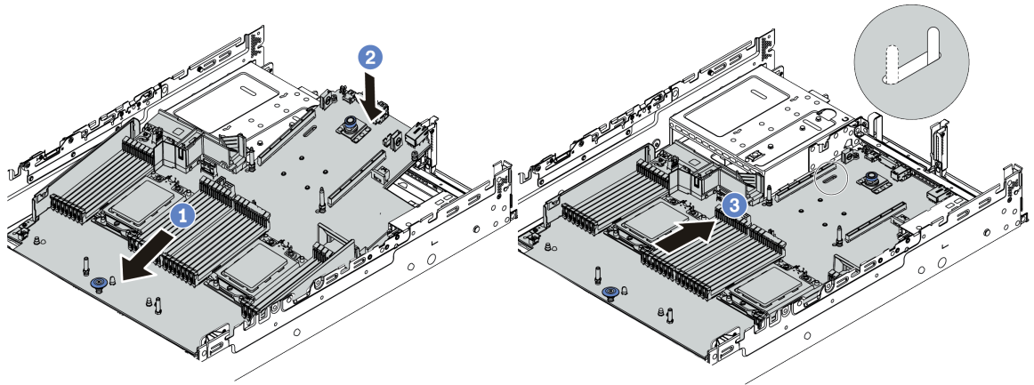
图 346. 安装主板
