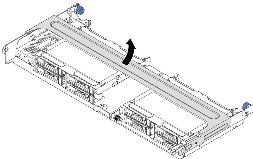
图 302. 打开中间硬盘仓的手柄
