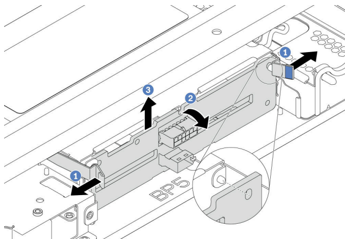
图 252. 卸下 2.5 英寸中间硬盘背板
