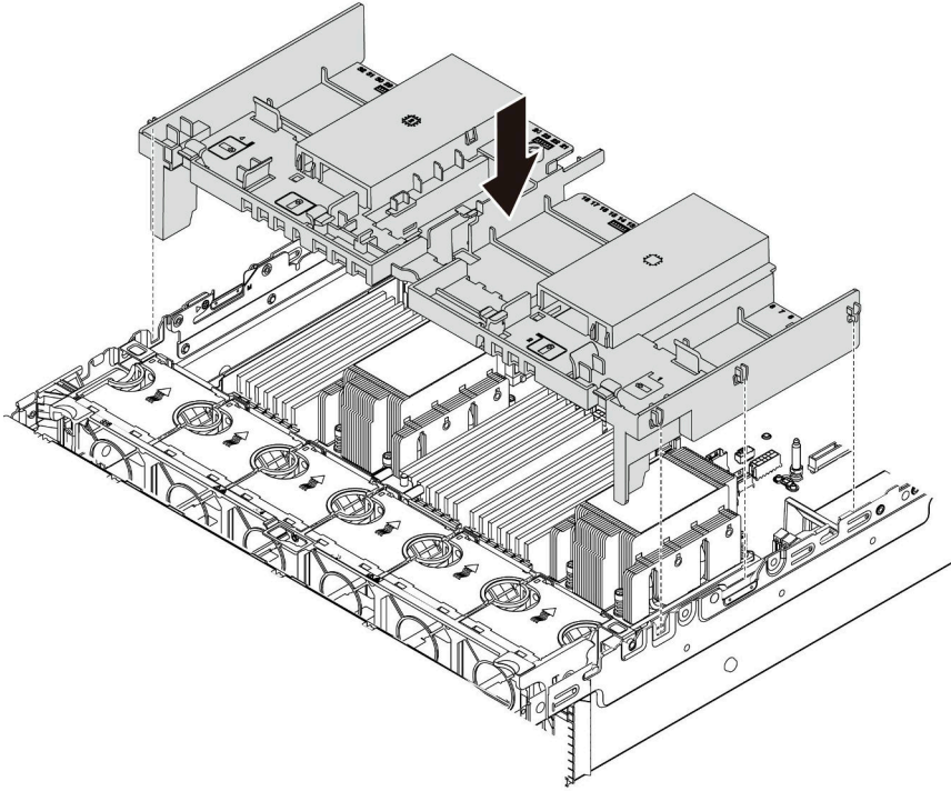
图 199. 安装标准导风罩
