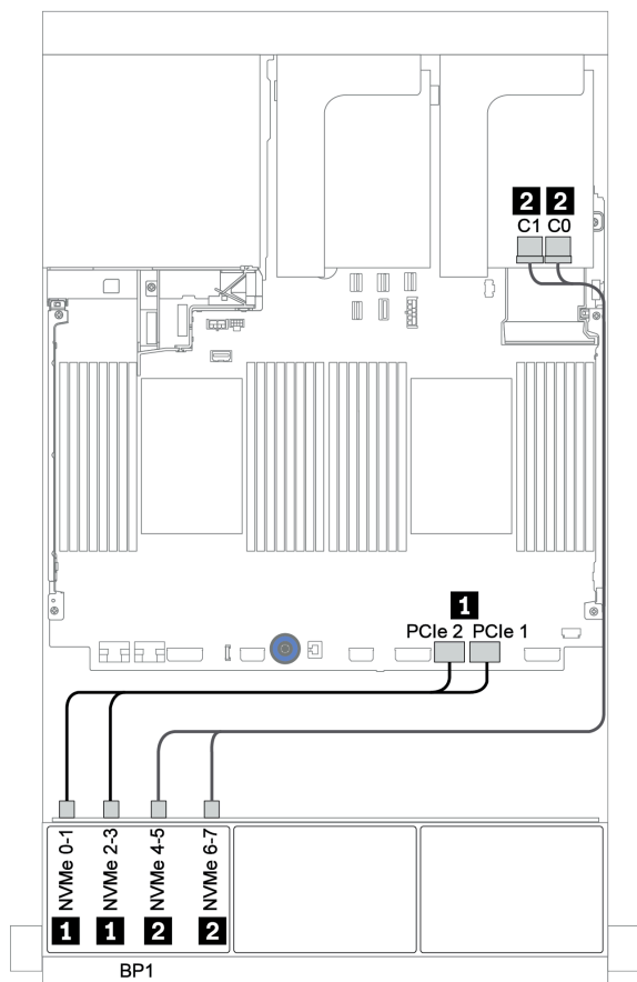
图 64. 配备一个重定时器卡的 8 x 2.5 英寸 NVMe 配置的线缆布放
