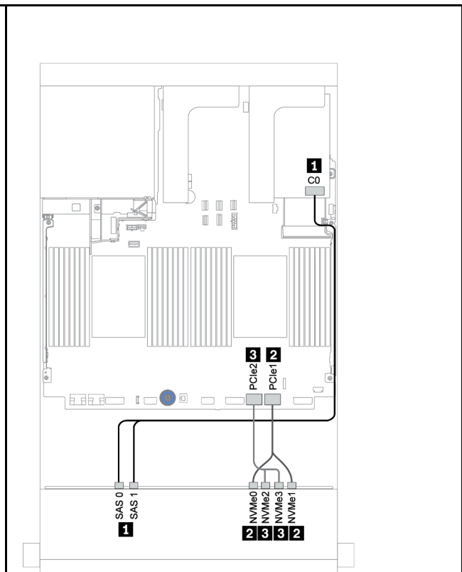
图 190. 配备 RAID 940-8i 适配器时的线缆布放
