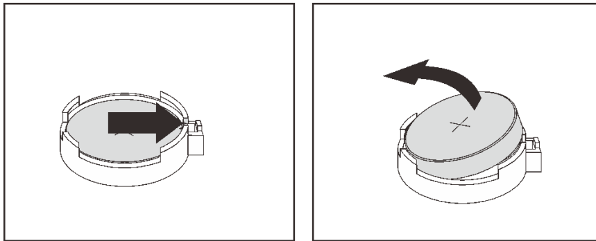
图 202. 卸下 CMOS 电池
