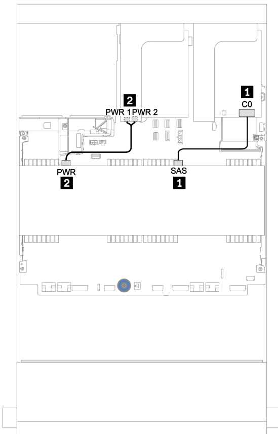
图 161. 4 x 3.5 英寸 SAS/SATA 中间背板的线缆布放
