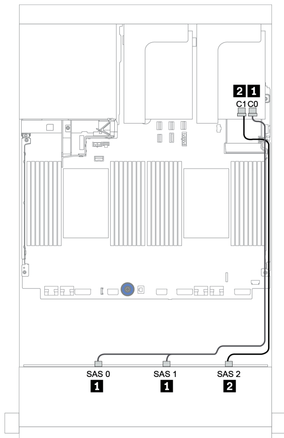
图 162. 配备一个 16i RAID/HBA 适配器的 12 x 3.5 英寸 SAS/SATA 正面背板的线缆布放
