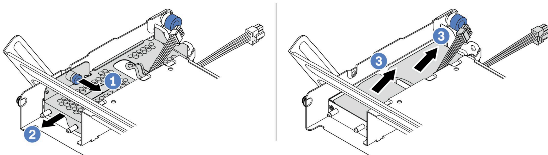
图 303. 卸下 RAID 快速充电模块
