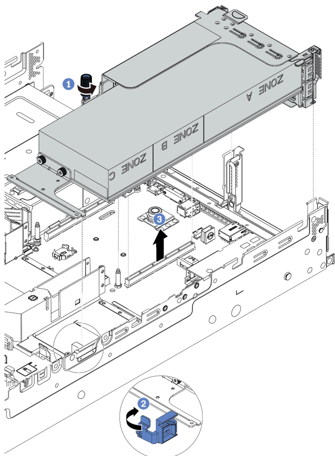
图 219. 卸下转接卡组合件
