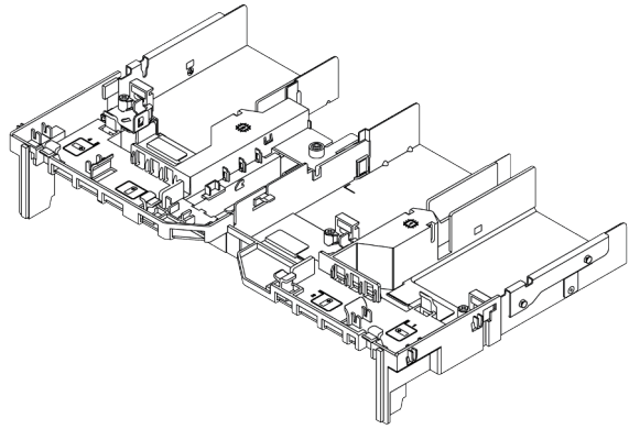
图 195. GPU 的导风罩
