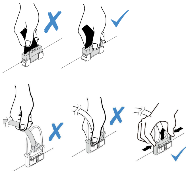
图 211. 拔下正面 I/O 模块线缆
