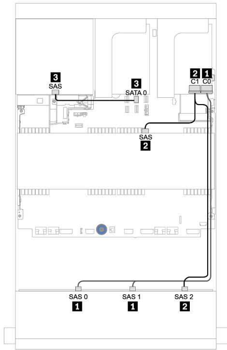
图 167. SAS/SATA 线缆布放
