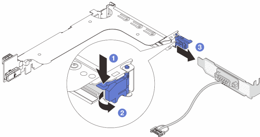
图 353. 卸下串口模块
