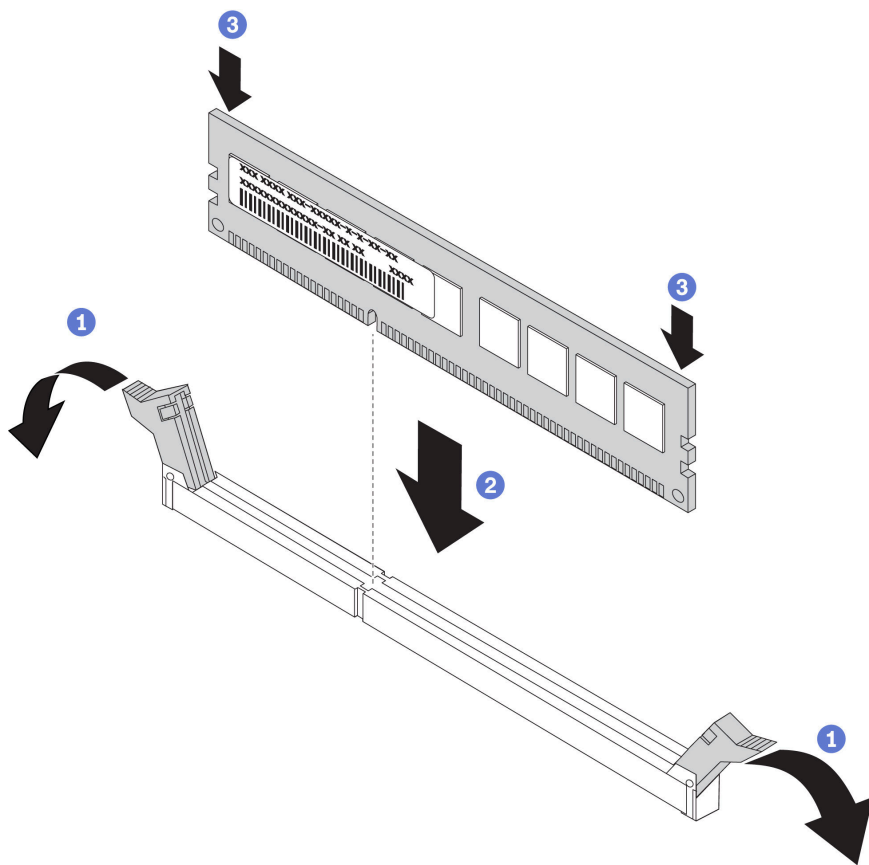
图 249. 安装内存条
