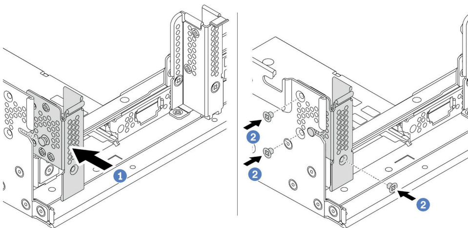
图 308. 安装 A1 后壁支架（左侧）
