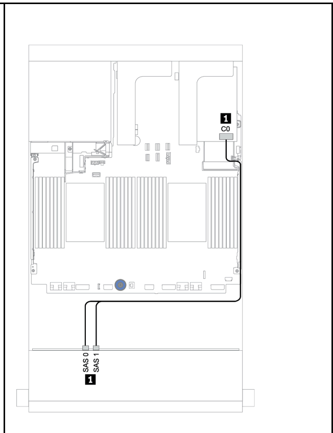
图 186. 配备 RAID 940-8i 适配器时的线缆布放
