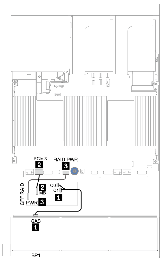
图 35. 配备一个 CFF 8i RAID 适配器的 8 x 2.5 英寸 SAS/SATA 配置的线缆布放
