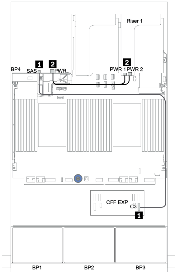
图 135. 4 x 2.5 英寸 SAS/SATA 背面背板的线缆布放
