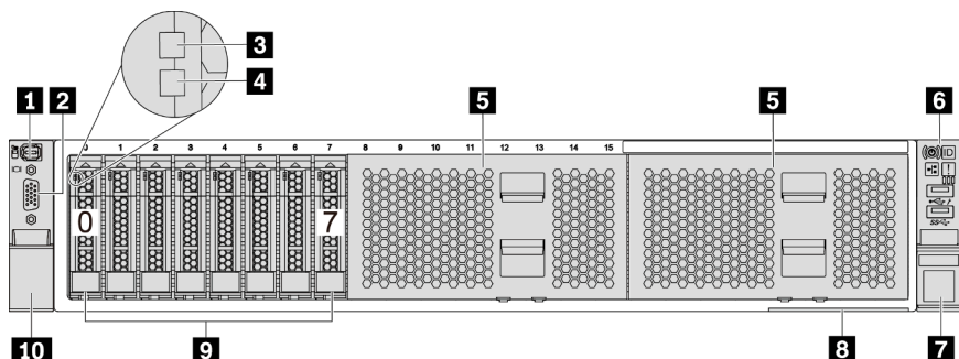
图 4. 配备八个 2.5 英寸正面硬盘插槽的服务器型号（型号 1）的前视图
