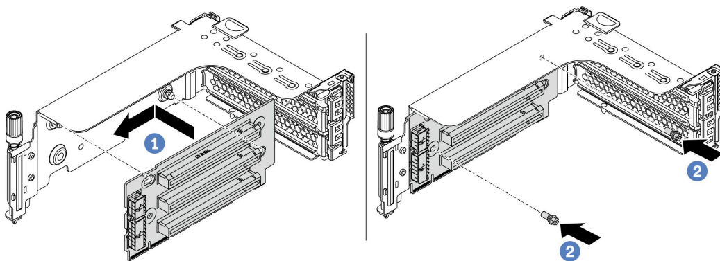
图 265. 安装转接卡
