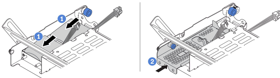
图 304. 安装 RAID 快速充电模块
