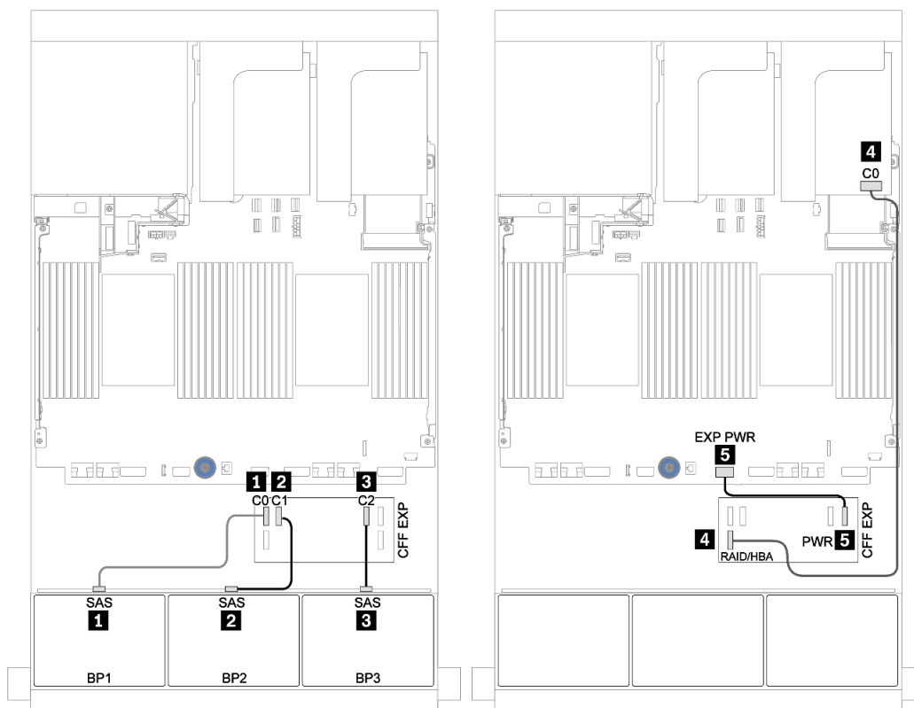
图 61. 配备一个 CFF 扩展器和一个 430/4350-16i 适配器的 24 x 2.5 英寸 SAS/SATA 配置的线缆布放
