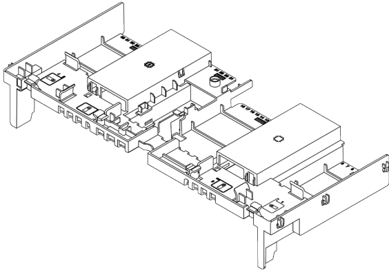
图 194. 标准导风罩
