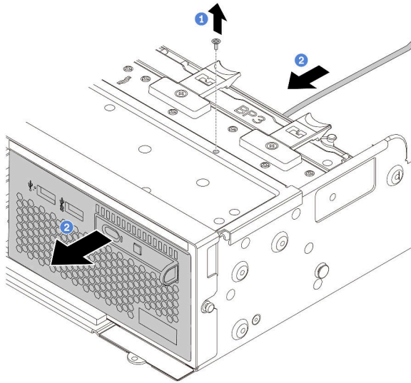
图 212. 卸下正面 I/O 模块
