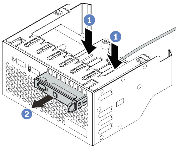
图 213. 卸下集成诊断面板
