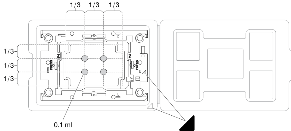
图 281. 为装运托盘中的处理器涂抹导热油脂
