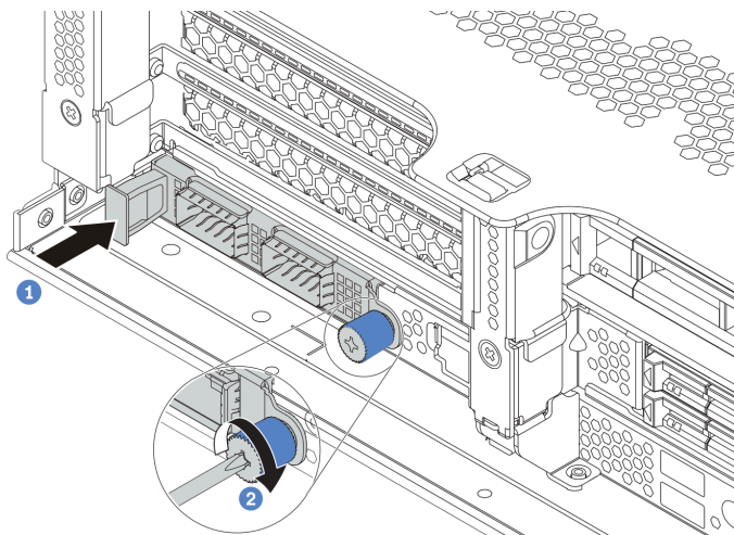
图 258. 安装 OCP 3.0 以太网适配器
