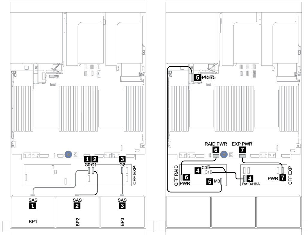
图 136. SAS/SATA 线缆布放
