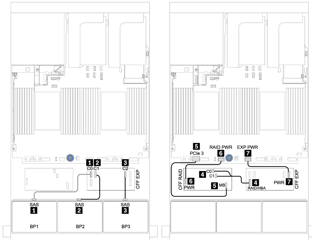
图 57. 配备一个 CFF 16i RAID/HBA 适配器和一个 CFF 扩展器的 24 x 2.5 英寸 SAS/SATA 配置的线缆布放
