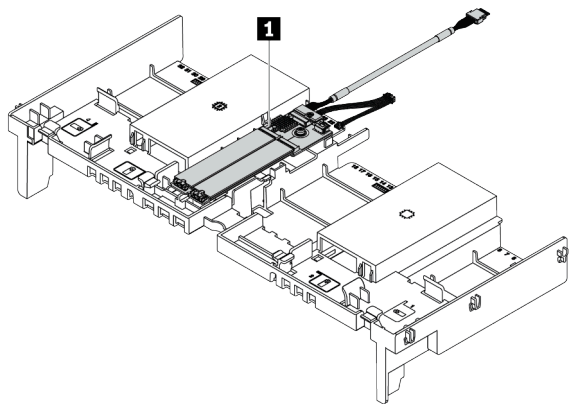
图 26. 在标准导风罩上
