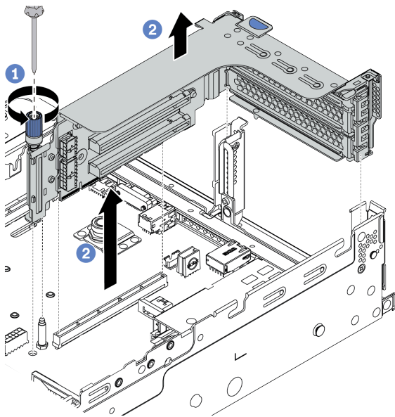
图 262. 卸下转接卡组合件
