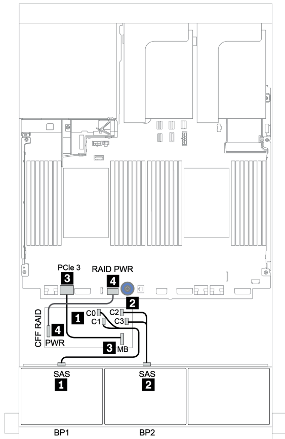
图 39. 配备一个 CFF 16i RAID/HBA 适配器的 16 x 2.5 英寸 SAS/SATA 配置的线缆布放
