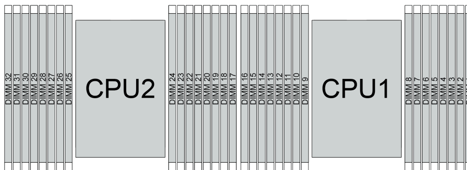
图 193. 主板上的内存条插槽
