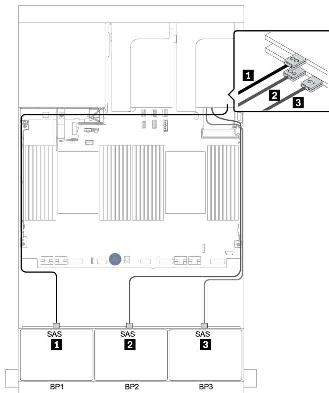
图 108. 配备一个 8i/16i RAID/HBA 适配器 和一个 三模式 16i RAID 适配器 的 8 x 2.5 英寸 SAS/SATA + 16 x 2.5 英寸 AnyBay 配置的线缆布放
