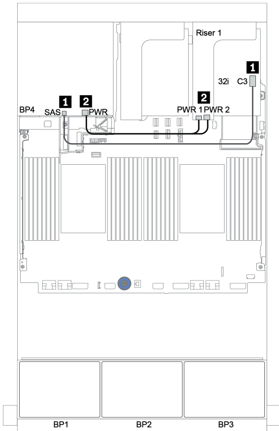
图 48. 4 x 2.5 英寸 SAS/SATA 背面背板的线缆布放
