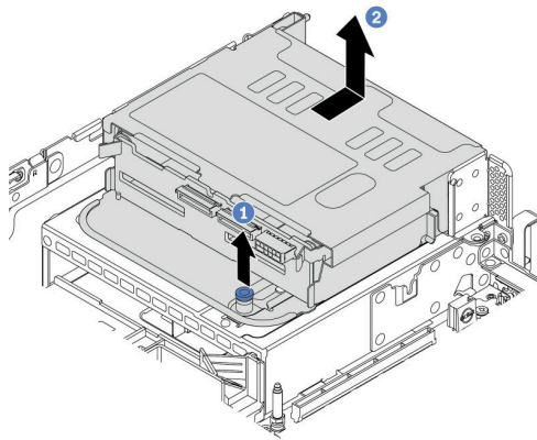
图 311. 卸下 4 x 2.5 英寸背面硬盘仓
