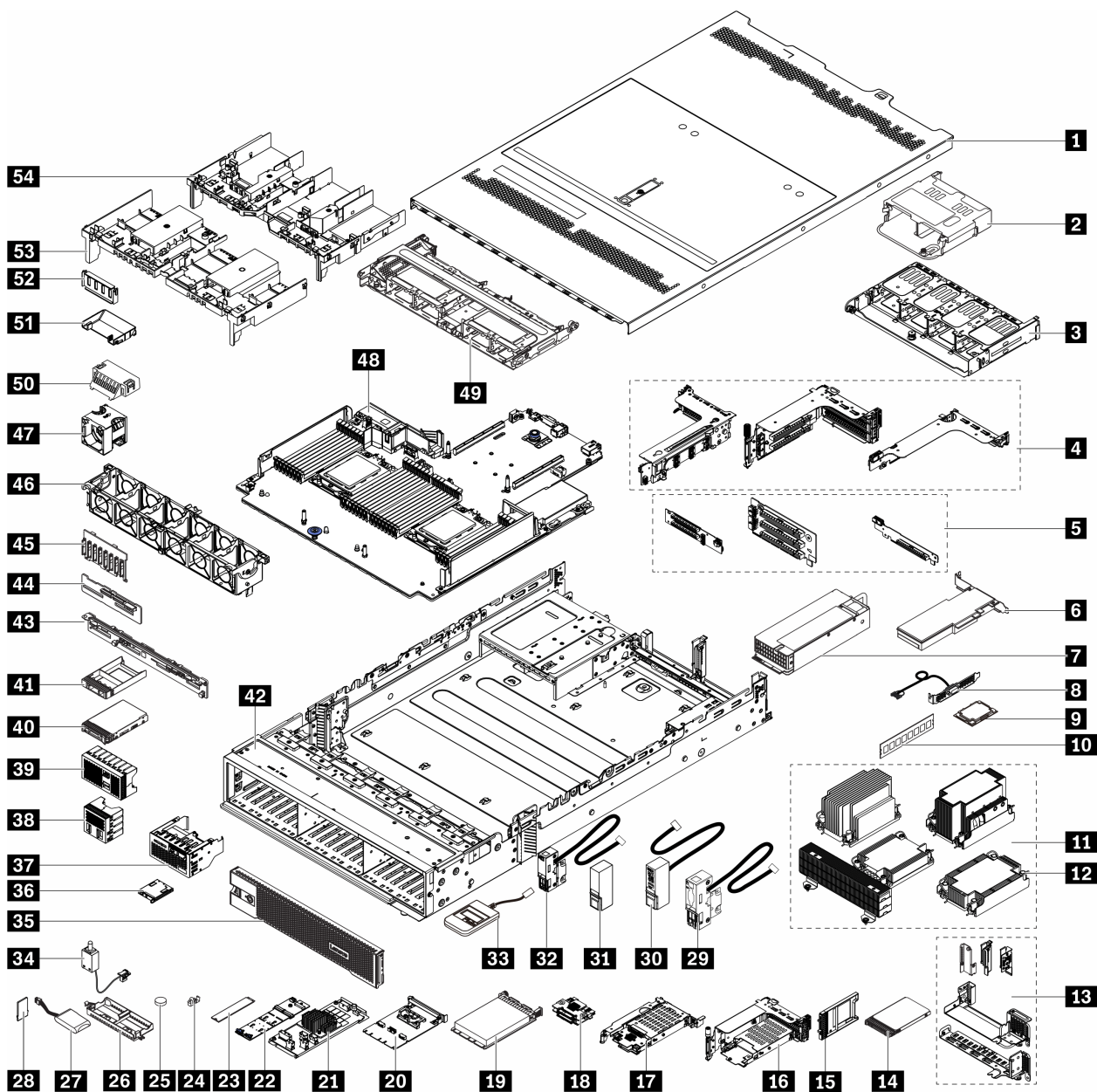
图 14. 服务器组件 (2.5 英寸硬盘插槽机箱)
