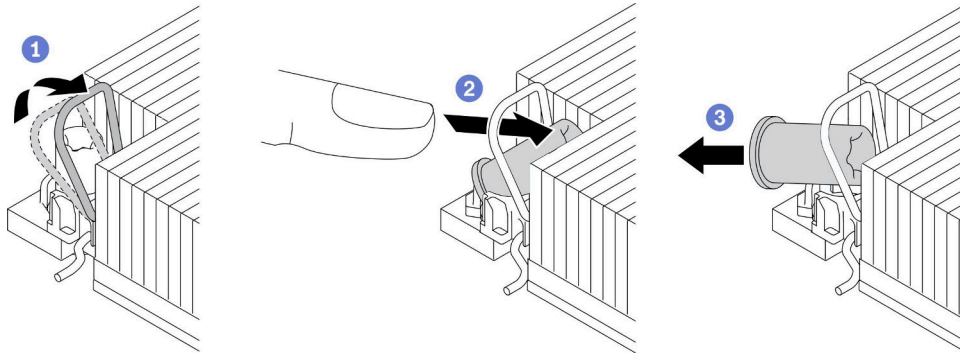
图 225. 从散热器上卸下内六角 T30 螺母
