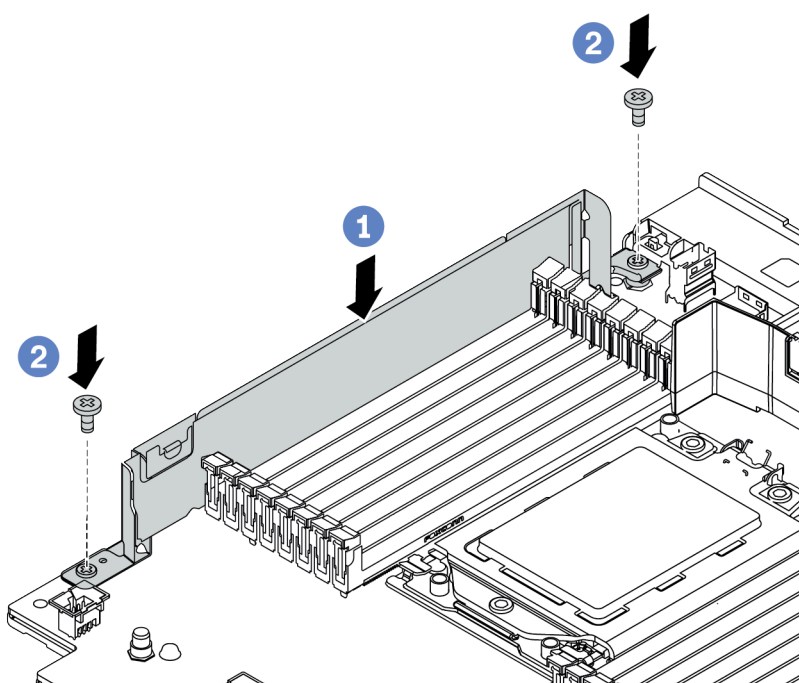
图 201. 安装线缆壁挂支架
