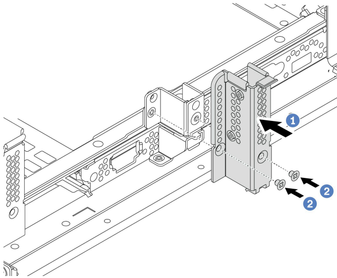
图 309. 安装 B1 后壁支架（中间）
