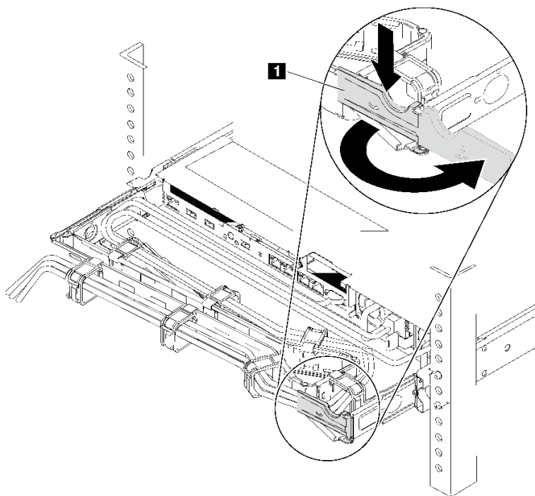
图 268. CMA 调整
