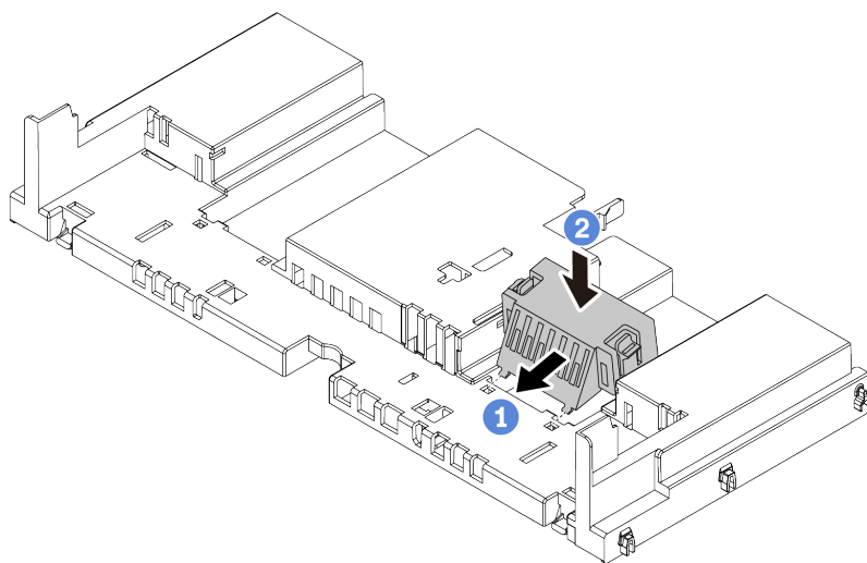
图 198. 安装导风罩填充件
