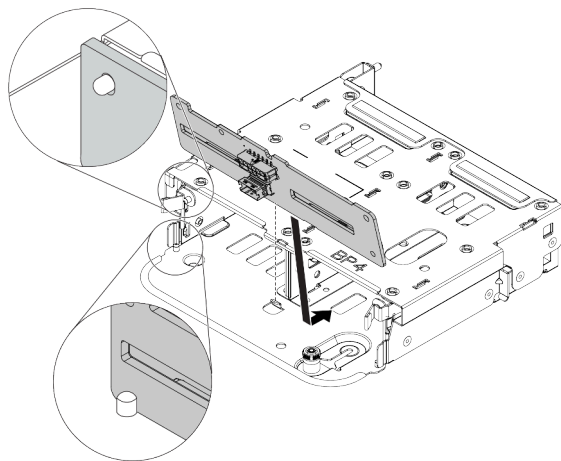
图 315. 安装 4 x 2.5 英寸背面硬盘背板
