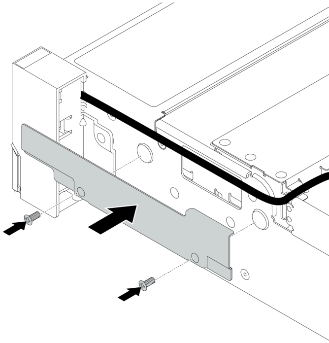
图 291. 安装线缆固定器
