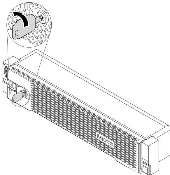
图 344. 锁定安全挡板
