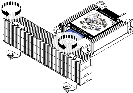
图 274. 拧松 T 形散热器的螺钉
