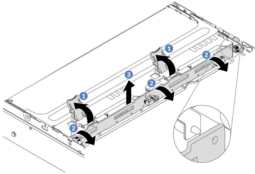
图 253. 卸下 3.5 英寸中间硬盘背板
