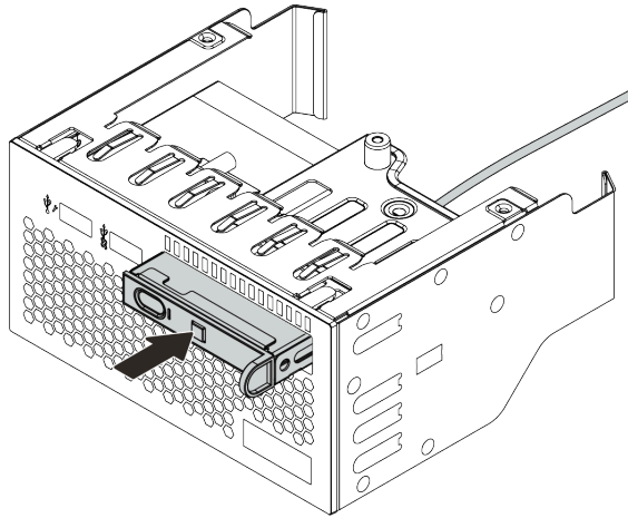
图 215. 安装集成诊断面板
