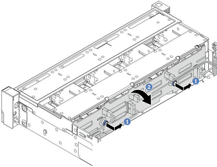
图 207. 卸下 3.5 英寸硬盘背板
