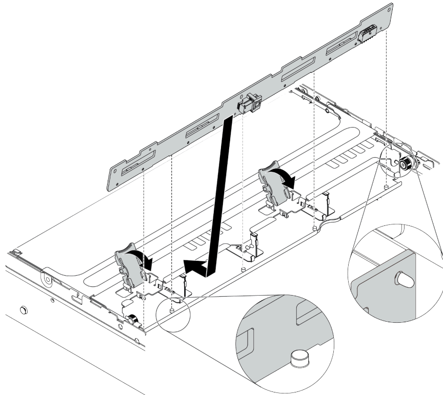
图 255. 安装 3.5 英寸中间硬盘背板
