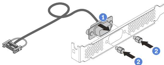
图 355. 组装串口模块
