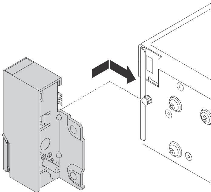
图 289. 安装机架滑锁
