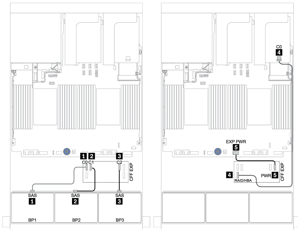
图 125. SAS/SATA 线缆布放
