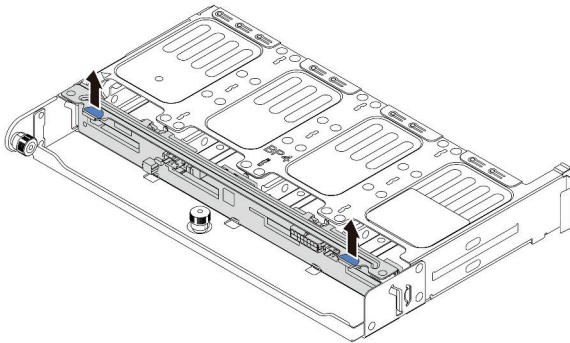
图 314. 卸下 8 x 2.5 英寸背面硬盘背板
