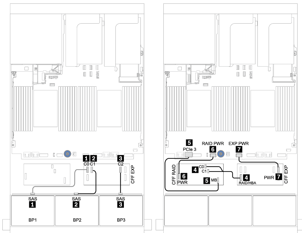
图 59. 配备一个 CFF 16i RAID/HBA 适配器和一个 CFF 扩展器的 24 x 2.5 英寸 SAS/SATA 配置的线缆布放
