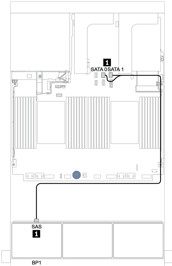
图 33. 配备板载接口的 8 x 2.5 英寸 SAS/SATA 配置的线缆布放
