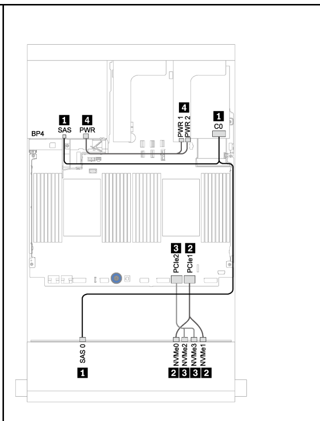
图 192. 配备 RAID 940-8i 适配器时的线缆布放
