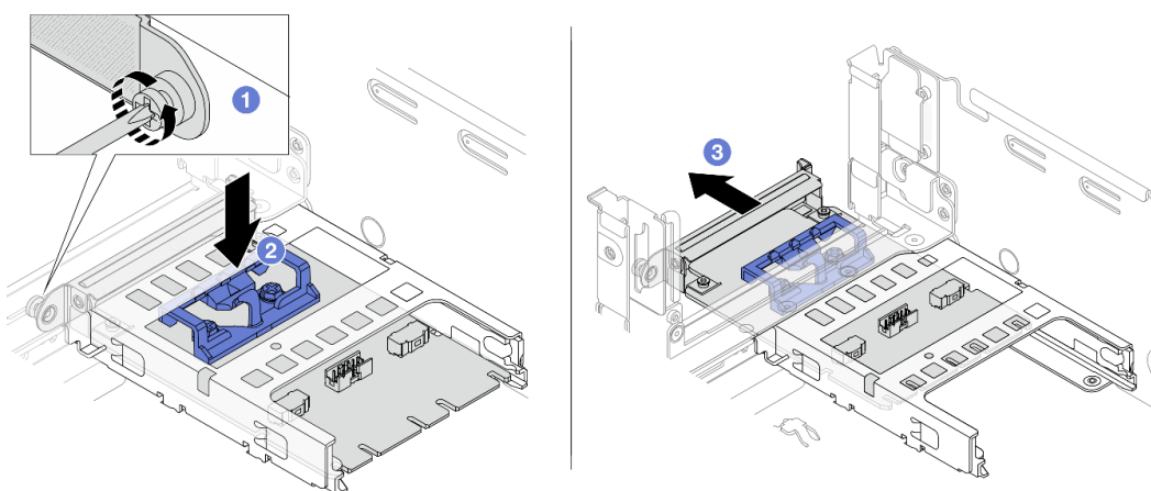
图 338. 卸下适用于 vSphere DSE 的 OCP 支持套件
