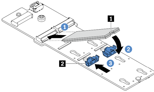
图 245. 安装 M.2 硬盘
