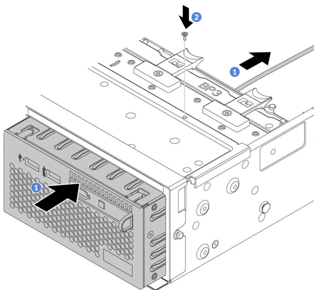
图 214. 安装正面 I/O 模块
