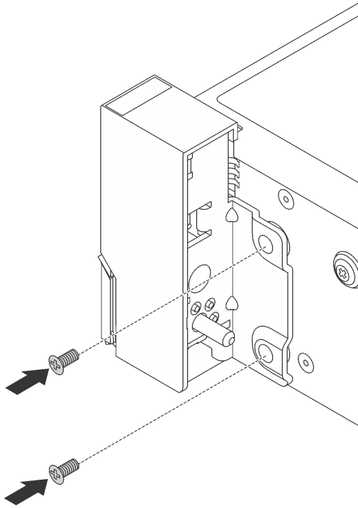
图 290. 螺钉安装
