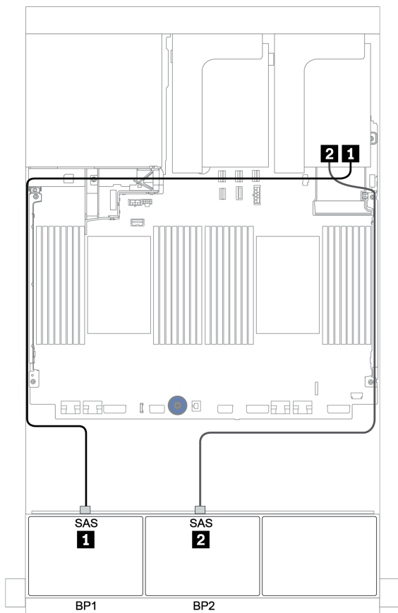
图 101. 配备一个 8i/16i RAID/HBA 适配器 和一个 三模式 8i RAID 适配器 的 8 x 2.5 英寸 SAS/SATA + 8 x 2.5 英寸 AnyBay 配置的线缆布放
