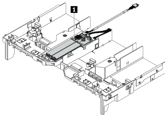
图 27. 在 GPU 导风罩上
