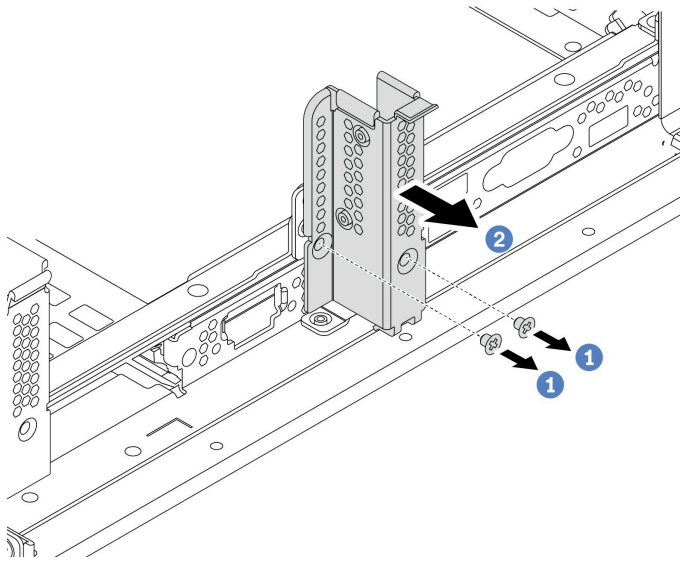
图 306. 卸下 B1 后壁支架（中间）
