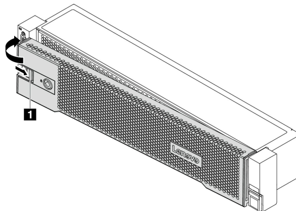
图 343. 安装安全挡板
