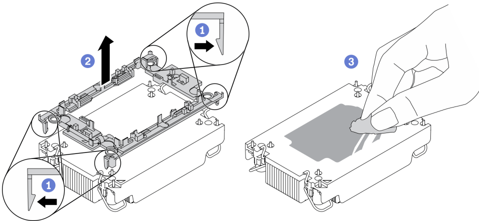
图 278. 将处理器支架与散热器分开
