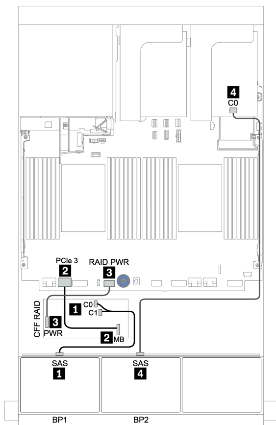
图 102. 配备一个 CFF 16i RAID/HBA 适配器和一个三模式 8i RAID 适配器的 8 x 2.5 英寸 SAS/SATA + 8 x 2.5 英寸 AnyBay 配置的线缆布放
