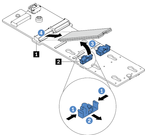
图 243. 卸下 M.2 硬盘
