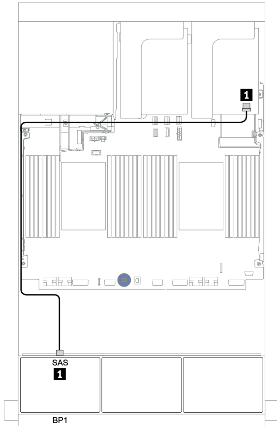
图 78. 配备一个三模式 8i RAID 适配器的 8 x 2.5 英寸 AnyBay 配置的线缆布放
