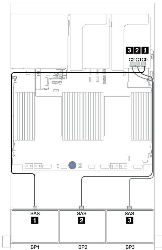
图 41. 配备一个 32i RAID 适配器的 24 x 2.5 英寸 SAS/SATA 配置的线缆布放
