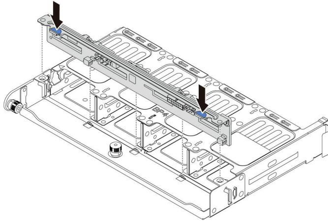
图 316. 安装 8 x 2.5 英寸背面硬盘背板
