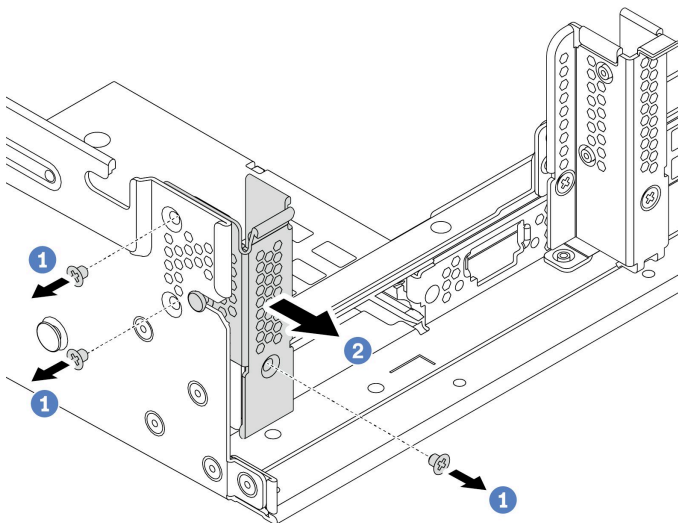
图 305. 卸下 A1 后壁支架（左侧）
