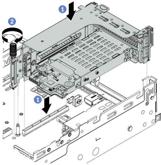
图 337. 安装转接卡组合件
