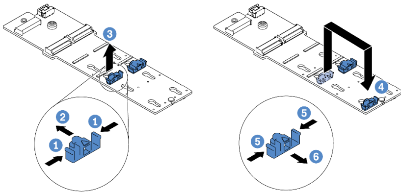
图 246. M.2 固定器调整
