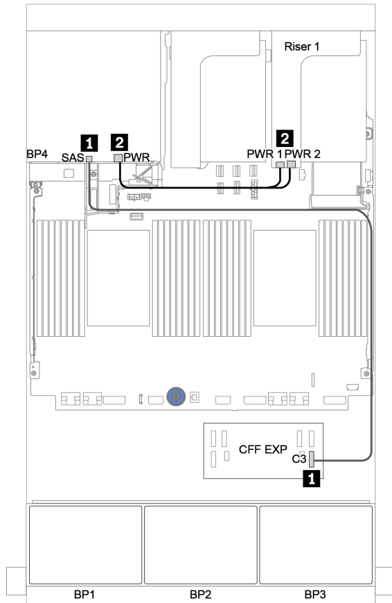
图 138. 4 x 2.5 英寸 SAS/SATA 背面背板的线缆布放
