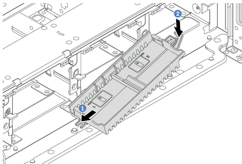
图 298. 安装超级电容器夹持器
