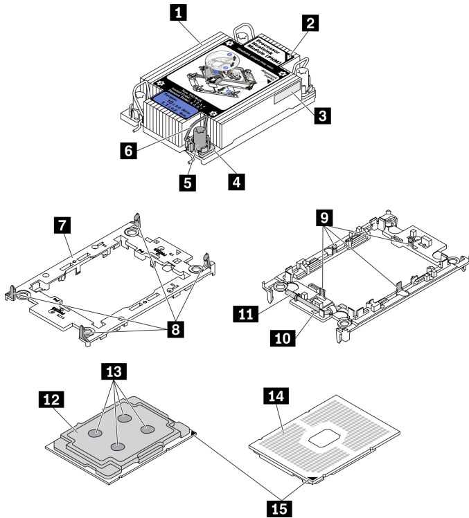
图 279. PHM 组件
