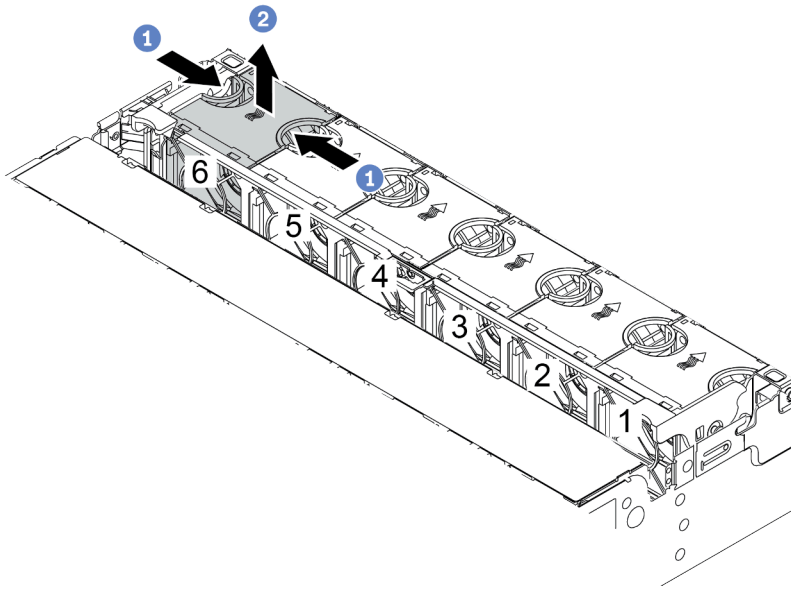
图 347. 卸下系统风扇
