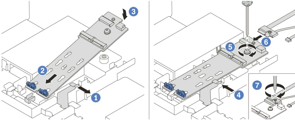
图 247. 安装 M.2 背板
