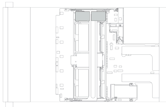
图 295. 在 2.5 英寸中间硬盘仓上
