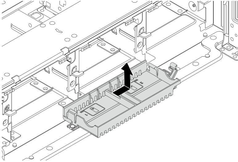
图 297. 卸下超级电容器夹持器
