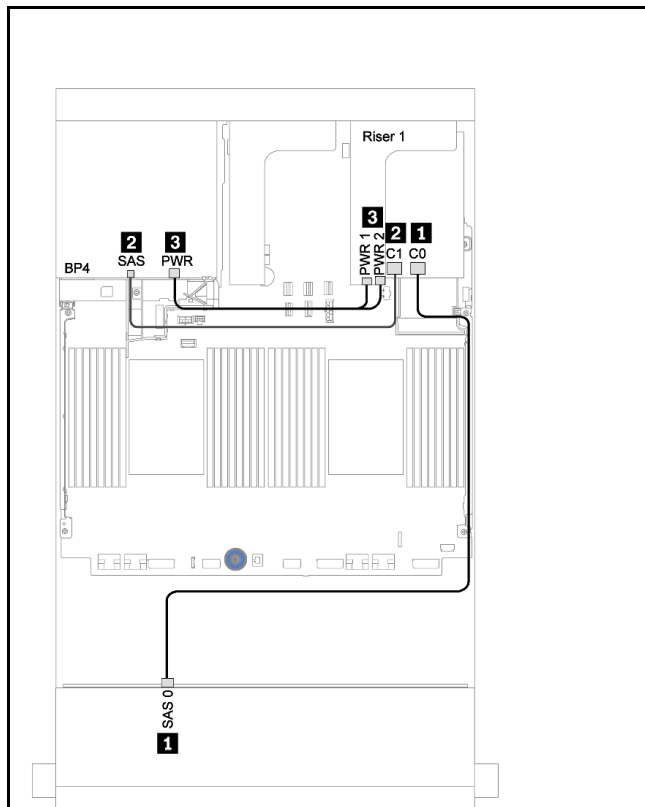
图 187. 配备 RAID 930/9350-8i 适配器时的线缆布放
