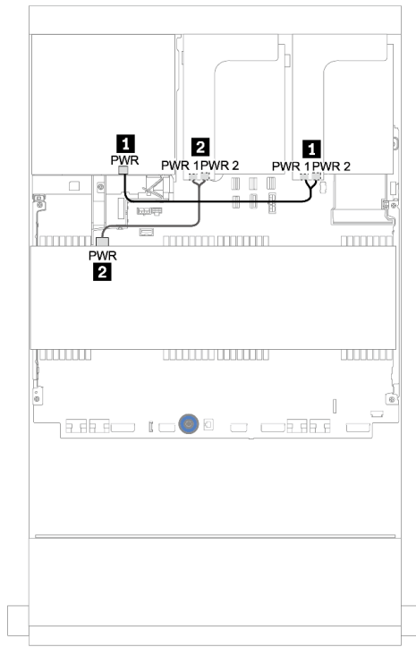
图 168. 电源线布放
