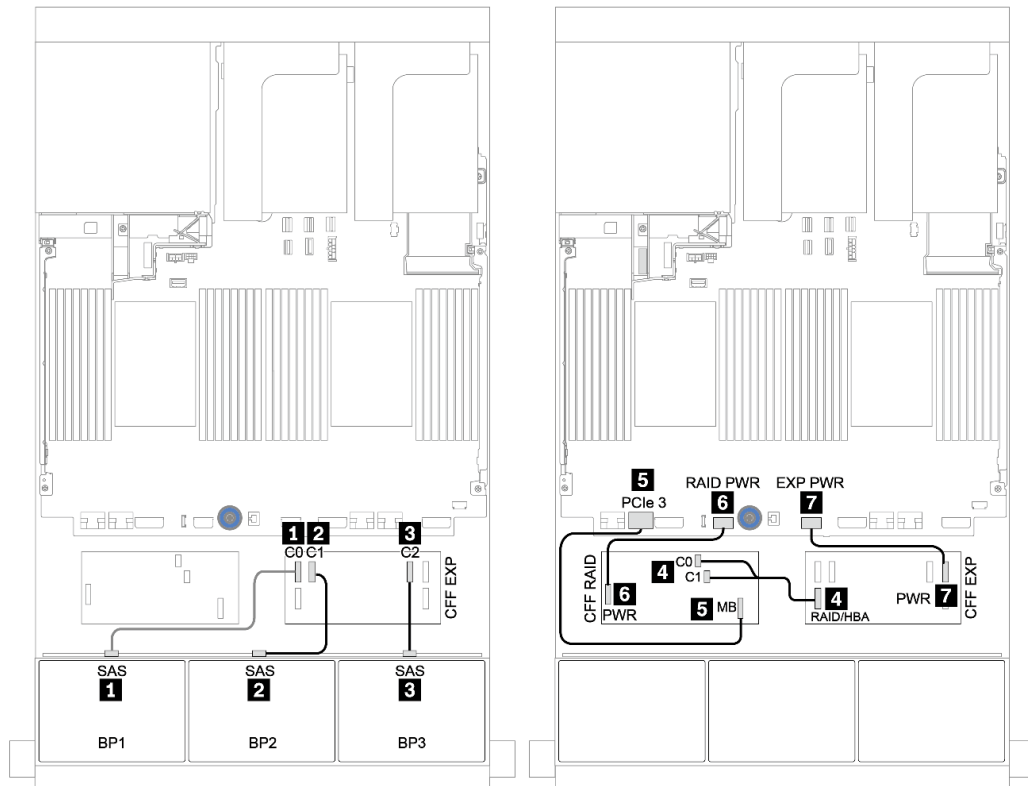
图 44. 配备一个 CFF 16i RAID/HBA 适配器和一个 CFF 扩展器的 24 x 2.5 英寸 SAS/SATA 配置的线缆布放
