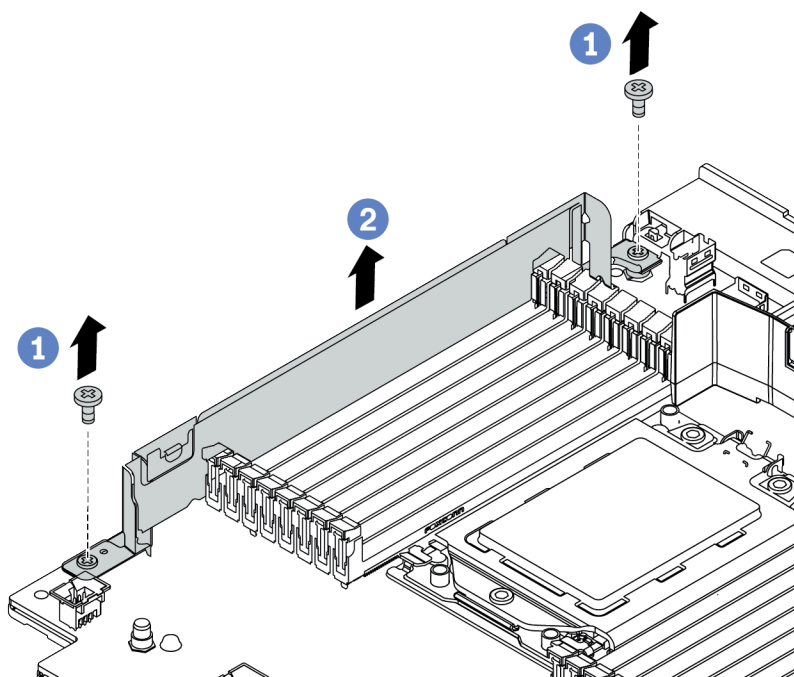
图 200. 卸下线缆壁挂支架
