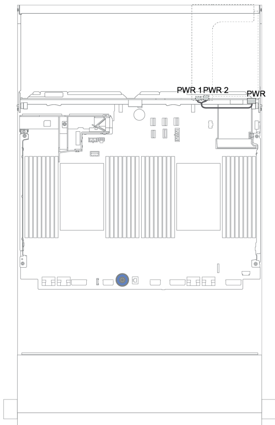
图 175. 背面背板的电源线布放
