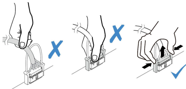
图 351. 拔下串口线缆
