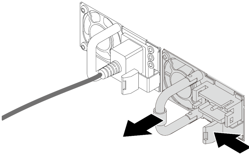
图 269. 卸下热插拔电源模块
