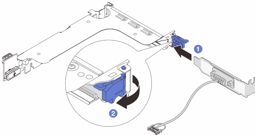
图 356. 安装串口模块
