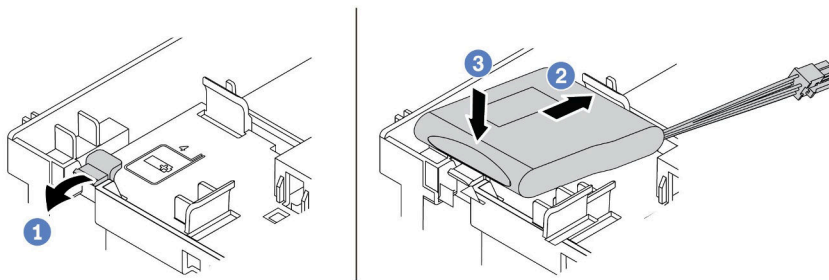
图 301. 将 RAID 快速充电模块安装在导风罩上
