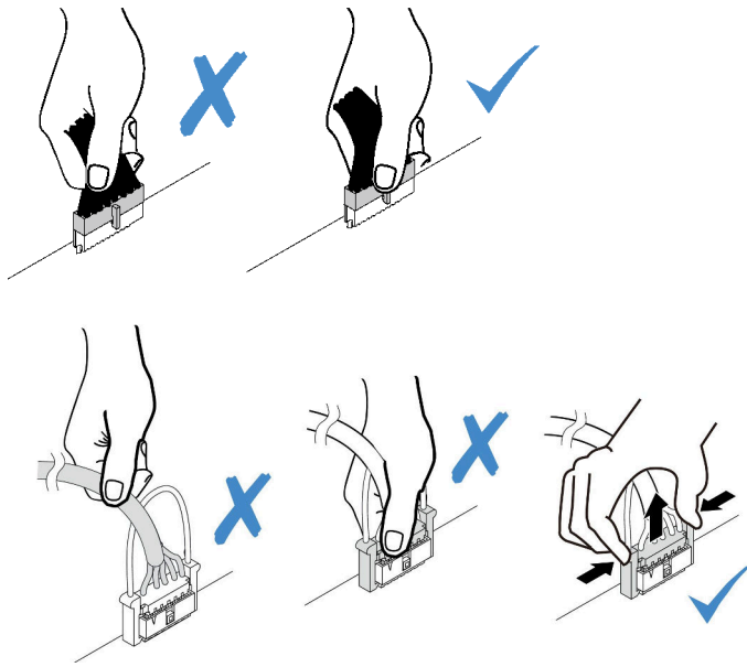
图 233. 从主板上拔下线缆
