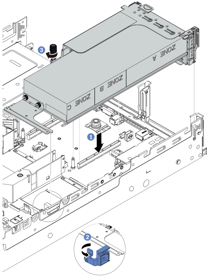
图 223. 安装转接卡组合件
