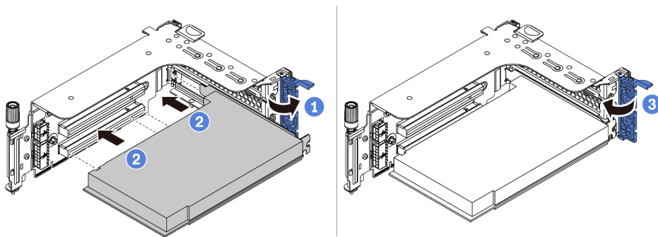
图 266. 安装 PCIe 适配器
