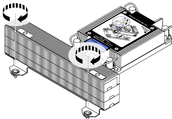
图 284. 拧紧 T 形散热器的螺钉
