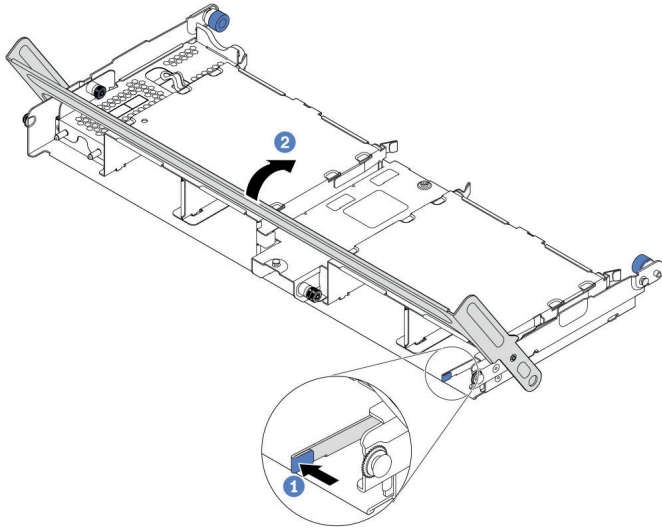
图 251. 合上硬盘仓手柄
