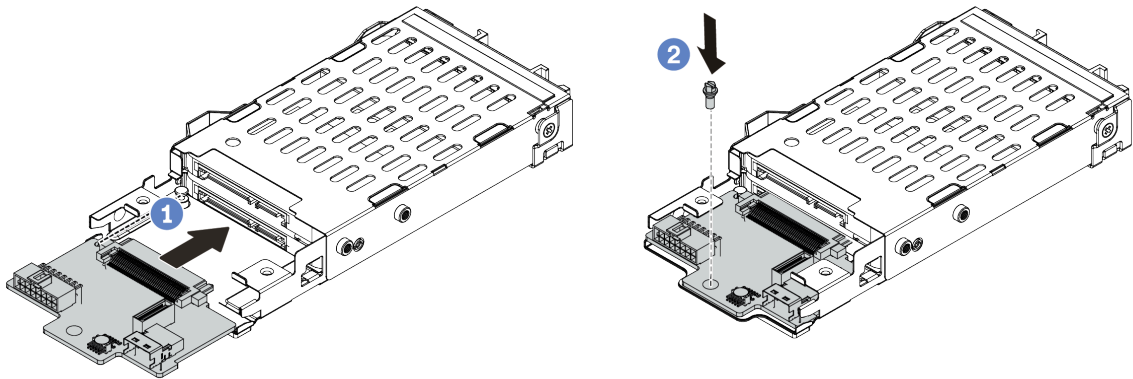
图 333. 安装 7 毫米硬盘背板（底部）
