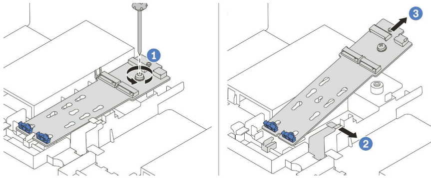
图 242. 卸下 M.2 背板
