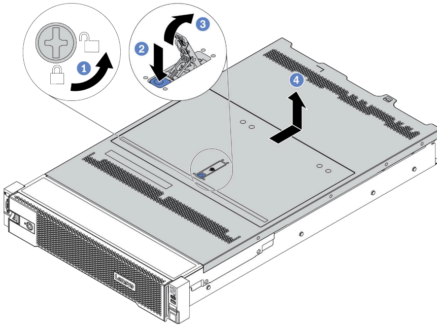
图 358. 卸下顶盖
