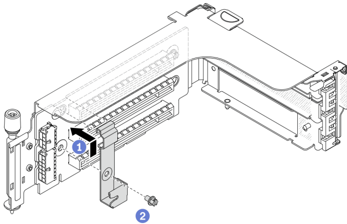
图 335. 安装 7 毫米硬盘仓固定夹
