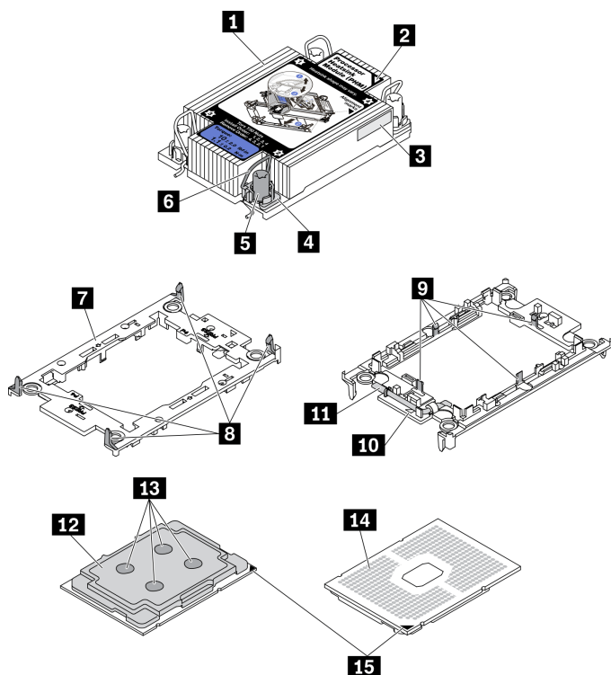
图 273. PHM 组件
