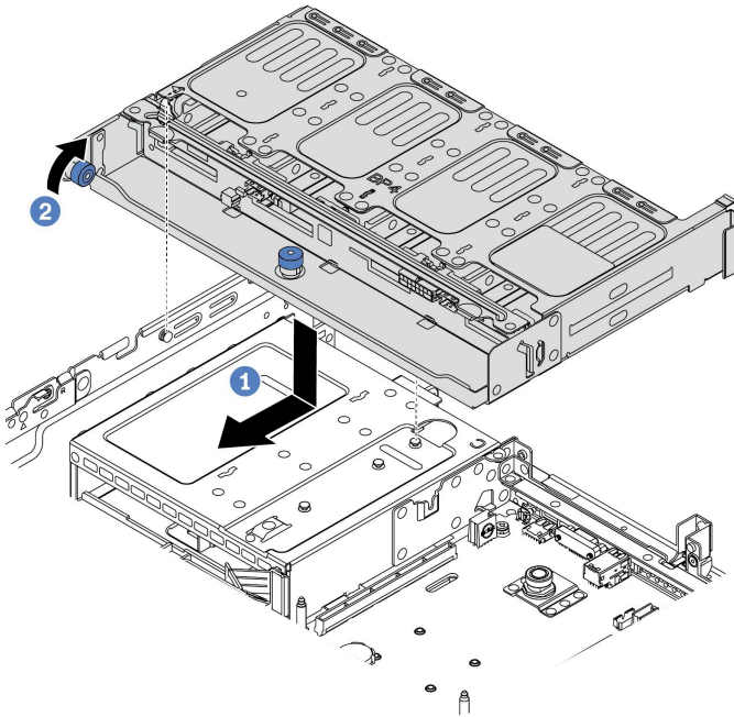
图 318. 安装 8 x 2.5 英寸背面硬盘仓
