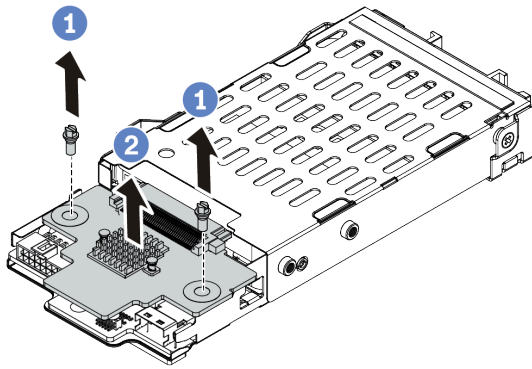
图 331. 7 毫米硬盘背板卸下 (顶部)
