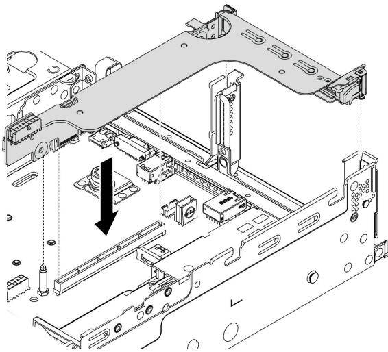
图 357. 安装转接卡组合件
