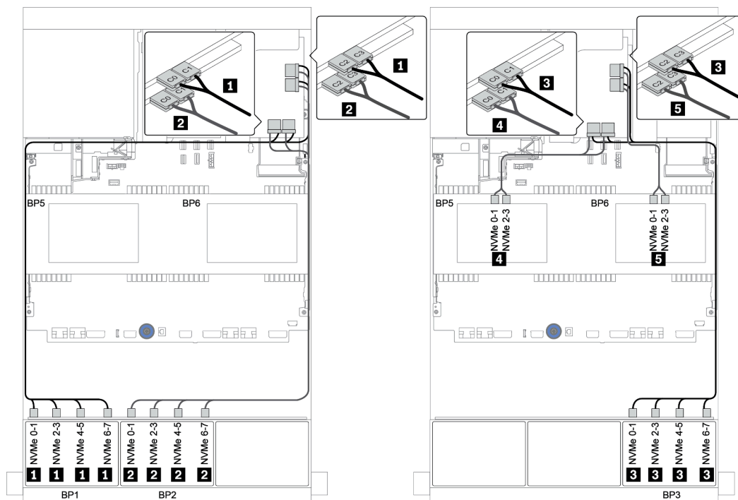
图 67. 配备四个交换卡的 32 x 2.5 英寸 NVMe 配置的线缆布局
