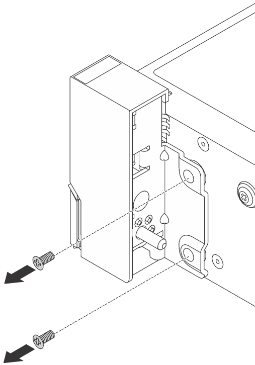
图 287. 卸下螺钉
