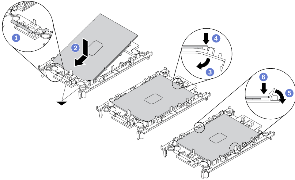
图 280. 安装处理器支架
