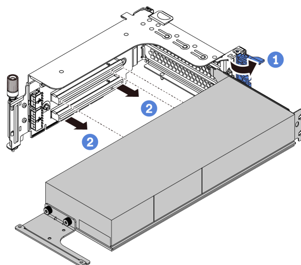
图 220. 卸下 GPU 适配器
