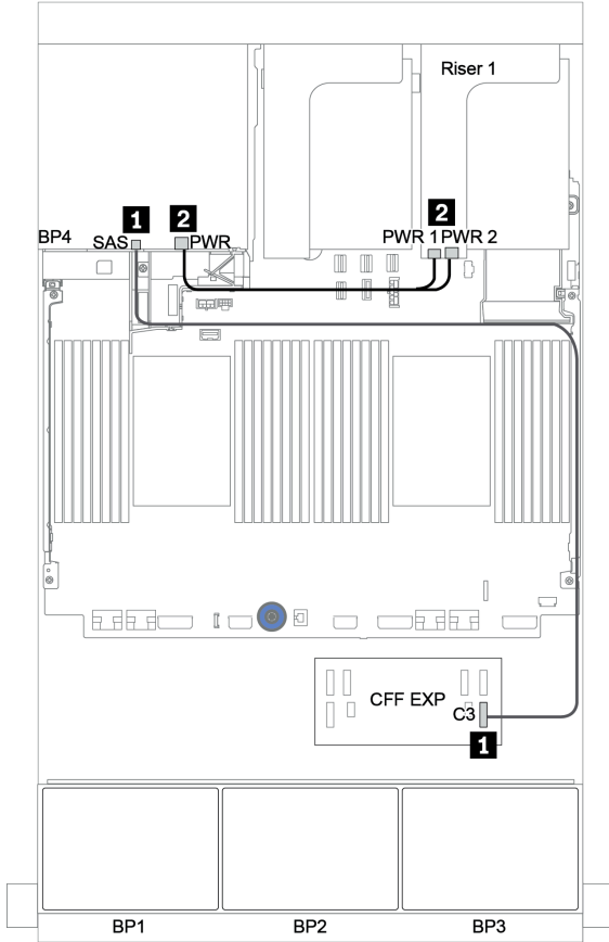
图 144. 4 x 2.5 英寸 SAS/SATA 背面背板的线缆布放
