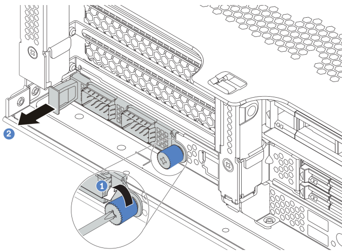
图 257. 卸下 OCP 3.0 以太网适配器
