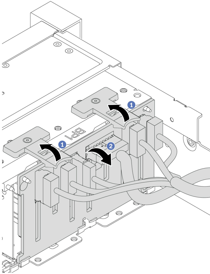
图 204. 卸下 2.5 英寸硬盘背板
