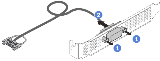
图 354. 拆卸串口模块
