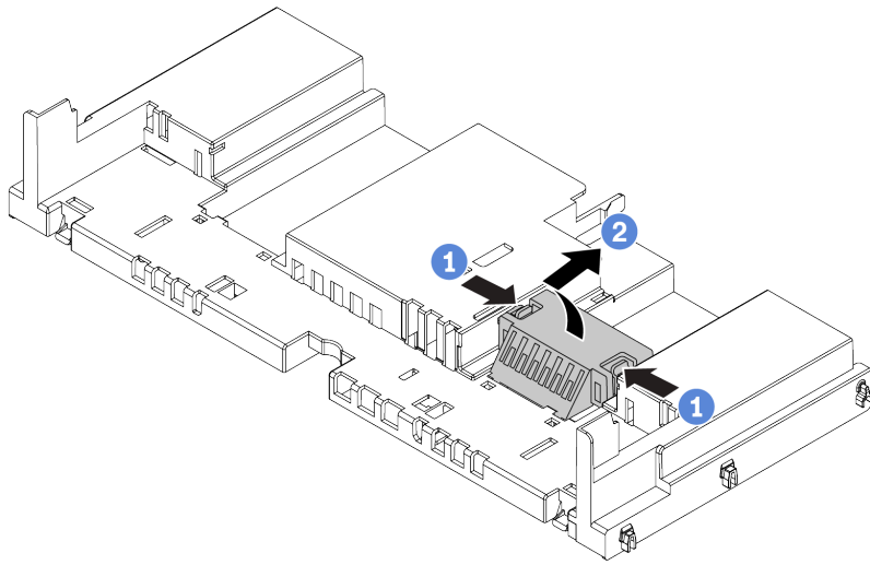
图 197. 卸下导风罩填充件
