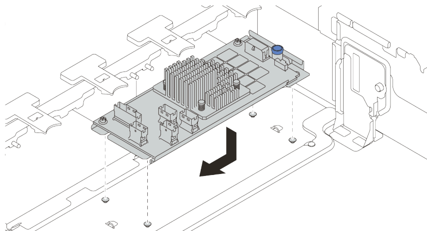
图 235. 安装内部 CFF 适配器
