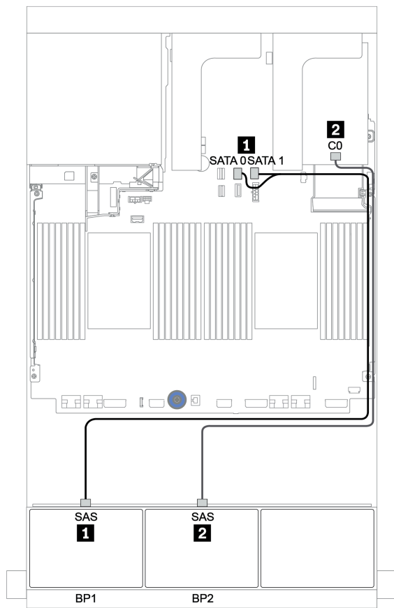
图 37. 配备一个 8i RAID 适配器的 16 x 2.5 英寸 SAS/SATA 配置的线缆布放
