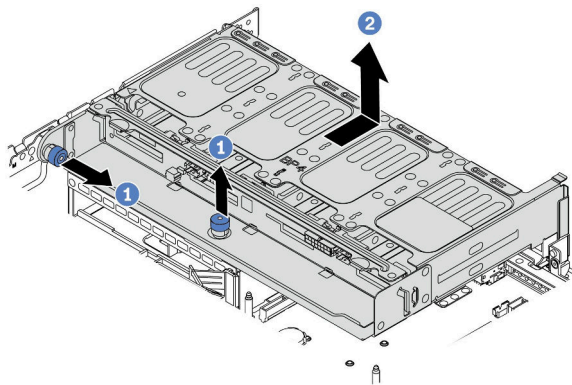
图 312. 卸下 8 x 2.5 英寸背面硬盘仓
