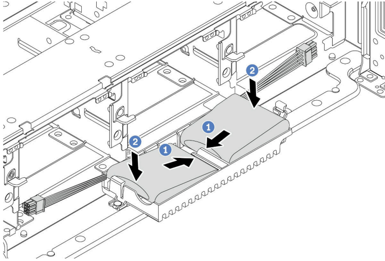
图 299. 安装 RAID 快速充电模块
