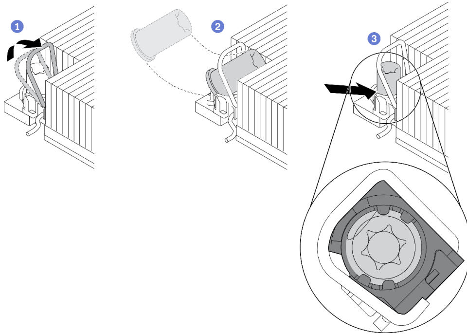
图 226. 将内六角 T30 螺母安装到散热器中
