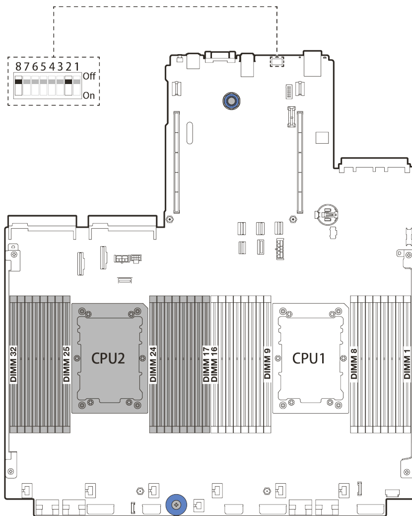
图 13. 主板上的 SW8 开关组
