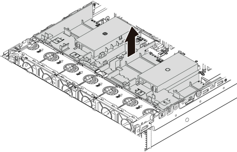
图 196. 卸下导风罩
