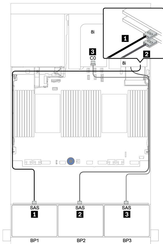
图 115. SAS/SATA 线缆布放
