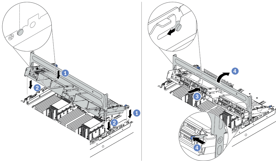
图 256. 安装中间硬盘仓和硬盘
