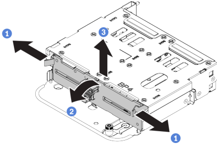
图 313. 卸下 4 x 2.5 英寸背面硬盘背板
