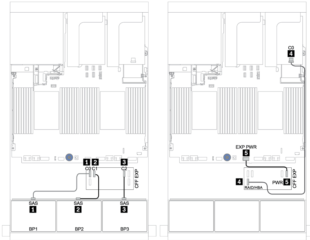
图 133. SAS/SATA 线缆布放
