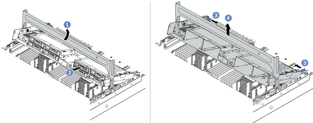
图 250. 卸下中间硬盘仓和硬盘
