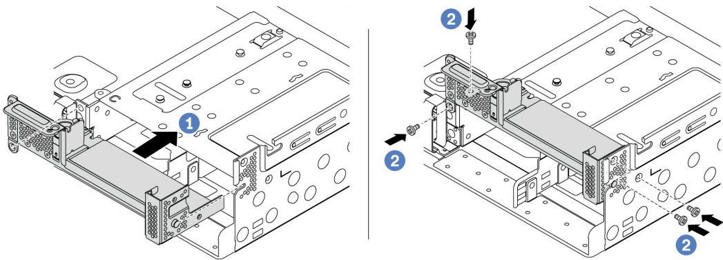
图 310. 安装 C1 后壁支架（右侧）
