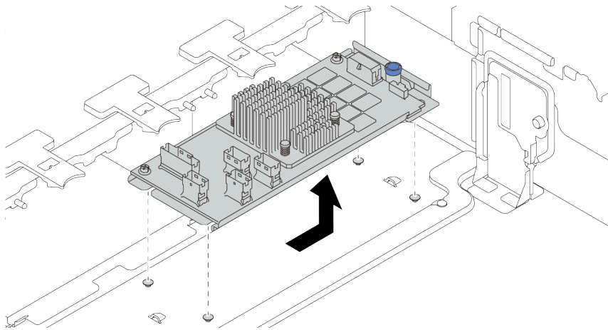
图 234. 卸下内部 CFF 适配器
