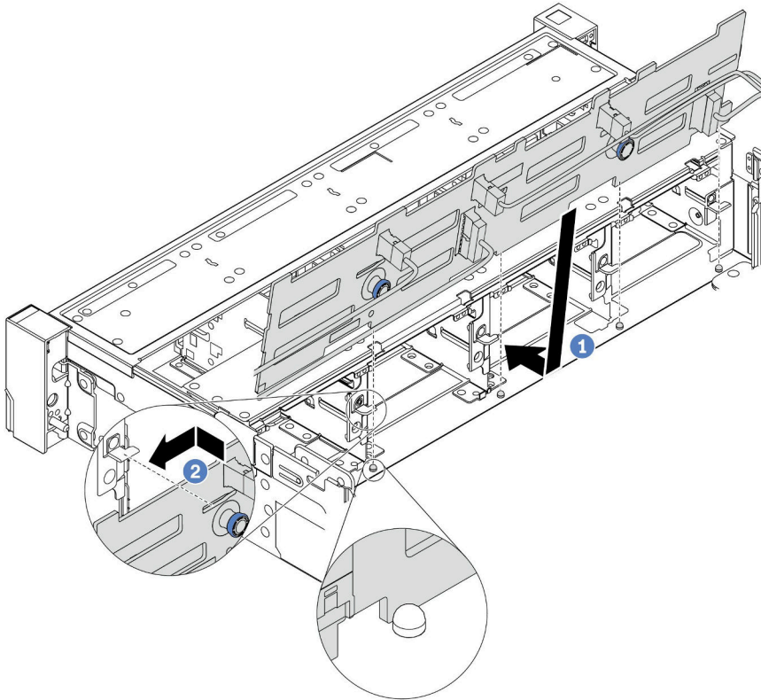
图 208. 安装 3.5 英寸硬盘背板
