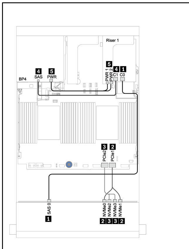
图 191. 配备 RAID 930/9350-8i 适配器时的线缆布放
