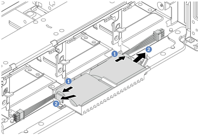
图 296. 卸下 RAID 快速充电模块
