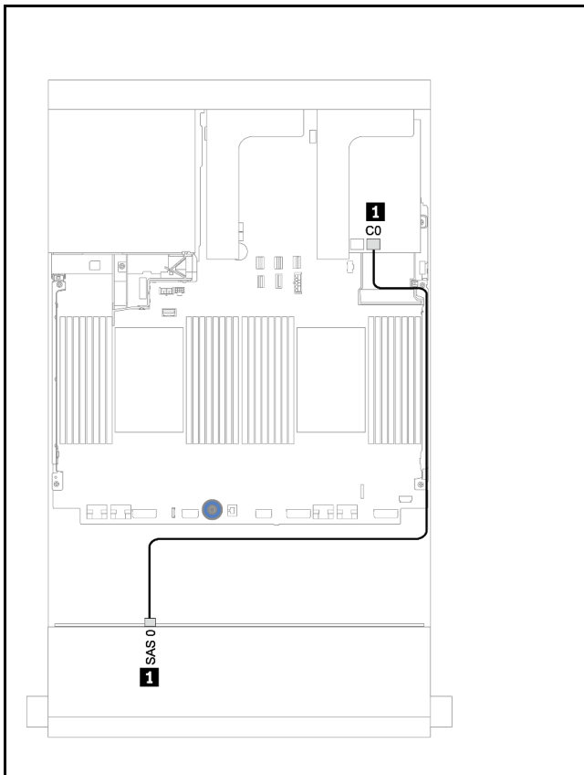
图 185. 配备 RAID 930/9350-8i 适配器时的线缆布放
