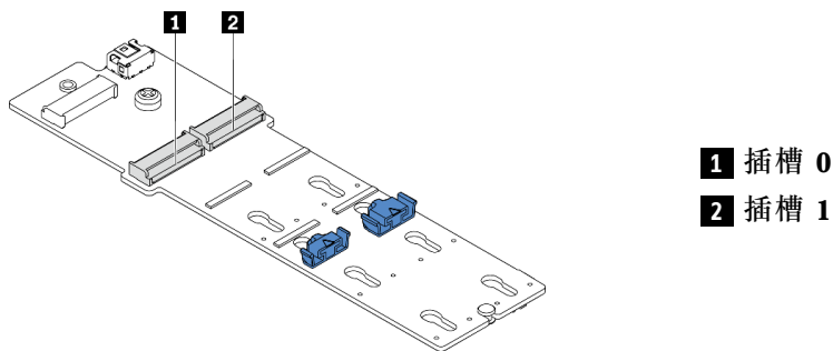
图 244. M.2 硬盘插槽
