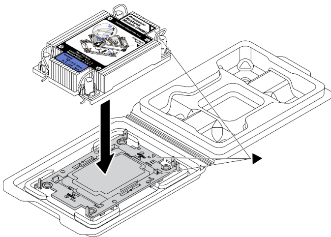
图 282. 在装运托盘中组装 PHM 和处理器
