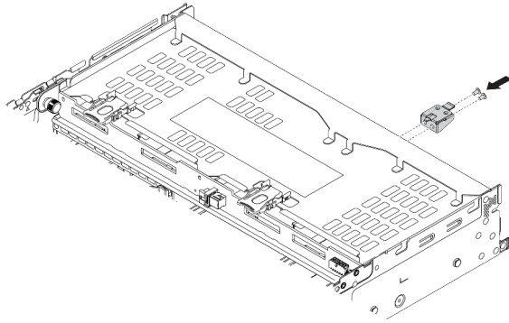
图 327. 安装顶盖支架
