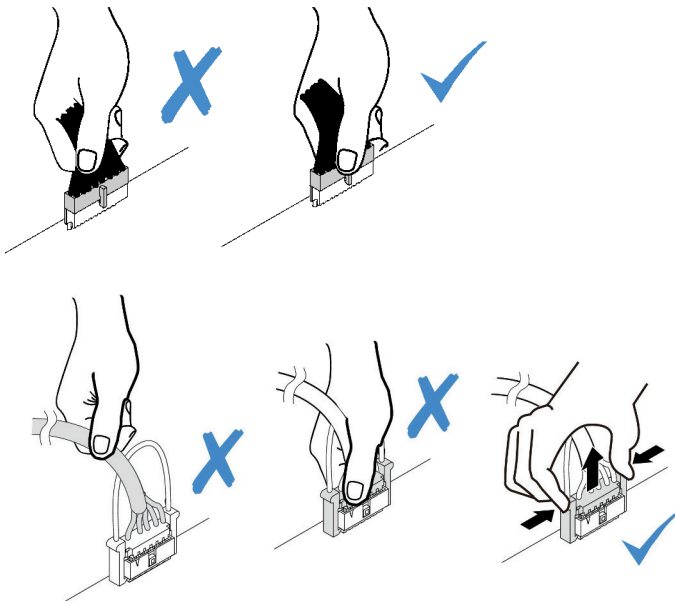
图 261. 从主板上拔下线缆
