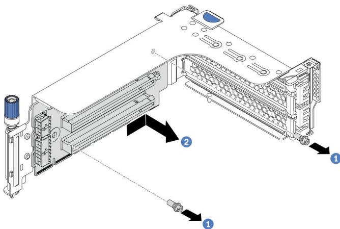
图 264. 卸下转接卡
