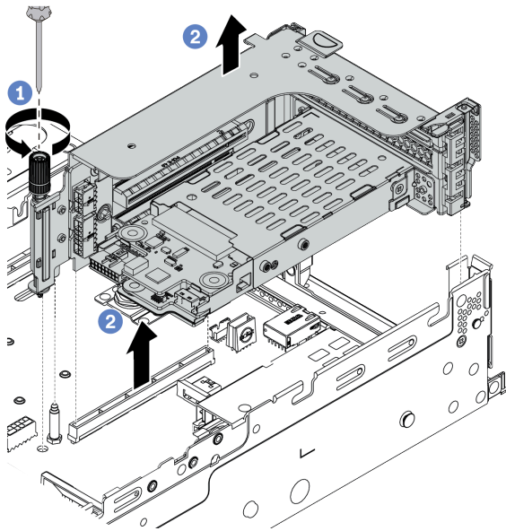
图 328. 卸下转接卡组合件
