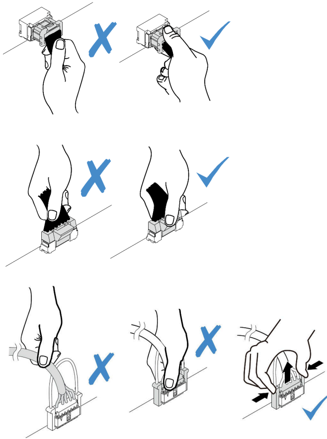
图 285. 从主板上拔下线缆
