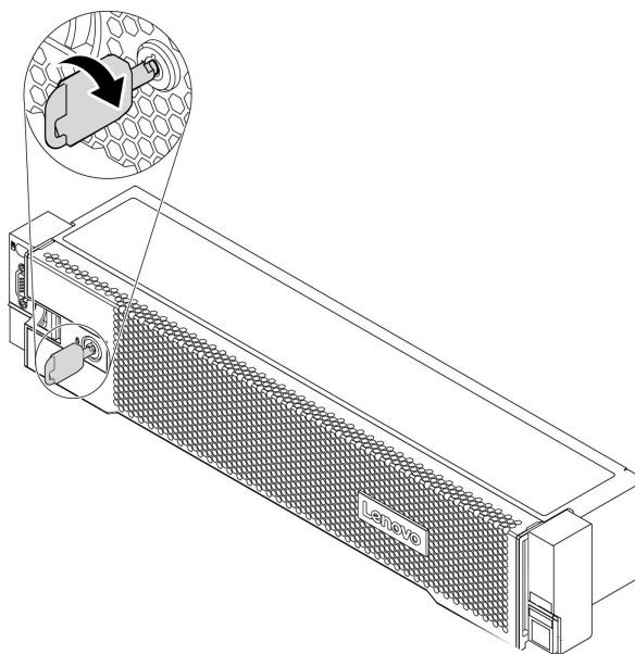
图 340. 解锁安全挡板
