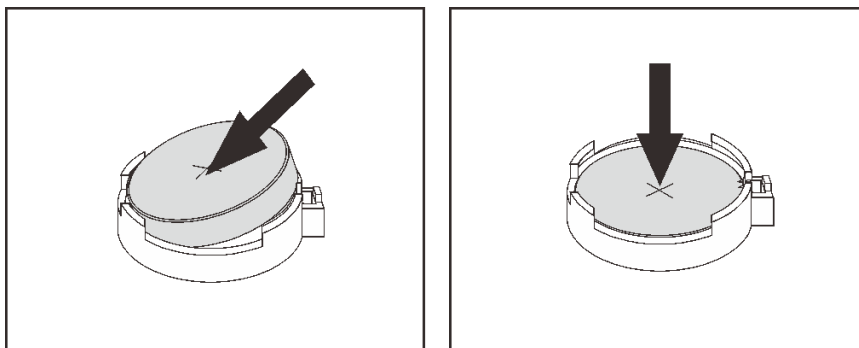
图 203. 安装 CMOS 电池
