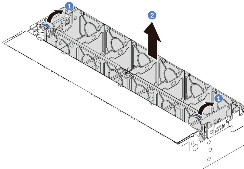
图 349. 卸下系统风扇架
