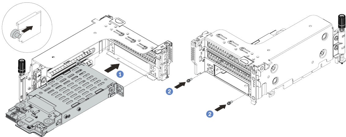
图 336. 安装 7 毫米硬盘仓
