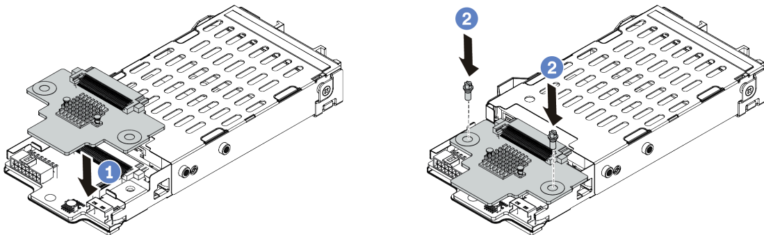
图 334. 安装 7 毫米硬盘背板 (顶部)
