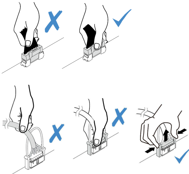
图 241. 从主板上拔下线缆
