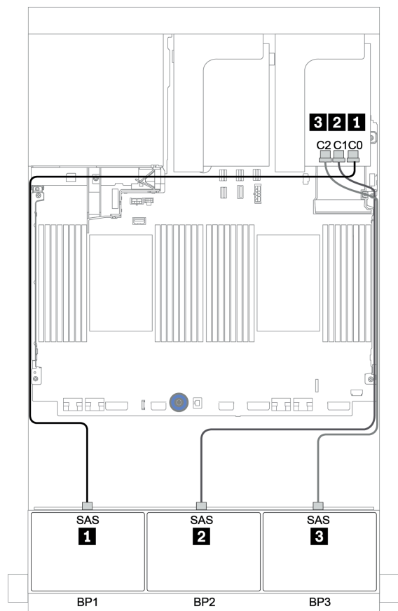
图 47. 配备一个 32i RAID 适配器的 24 x 2.5 英寸 SAS/SATA 配置的线缆布放
