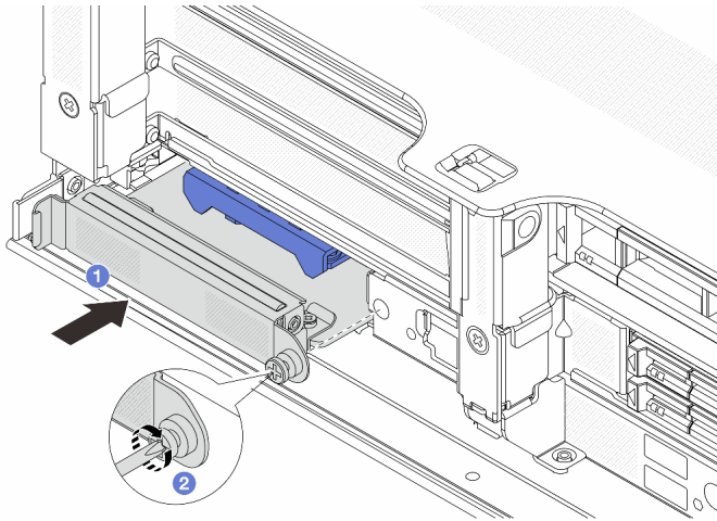
图 339. 安装适用于 vSphere DSE 的 OCP 支持套件
