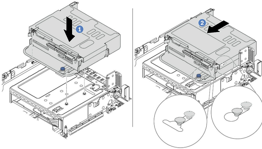
图 317. 安装 4 x 2.5 英寸背面硬盘仓
