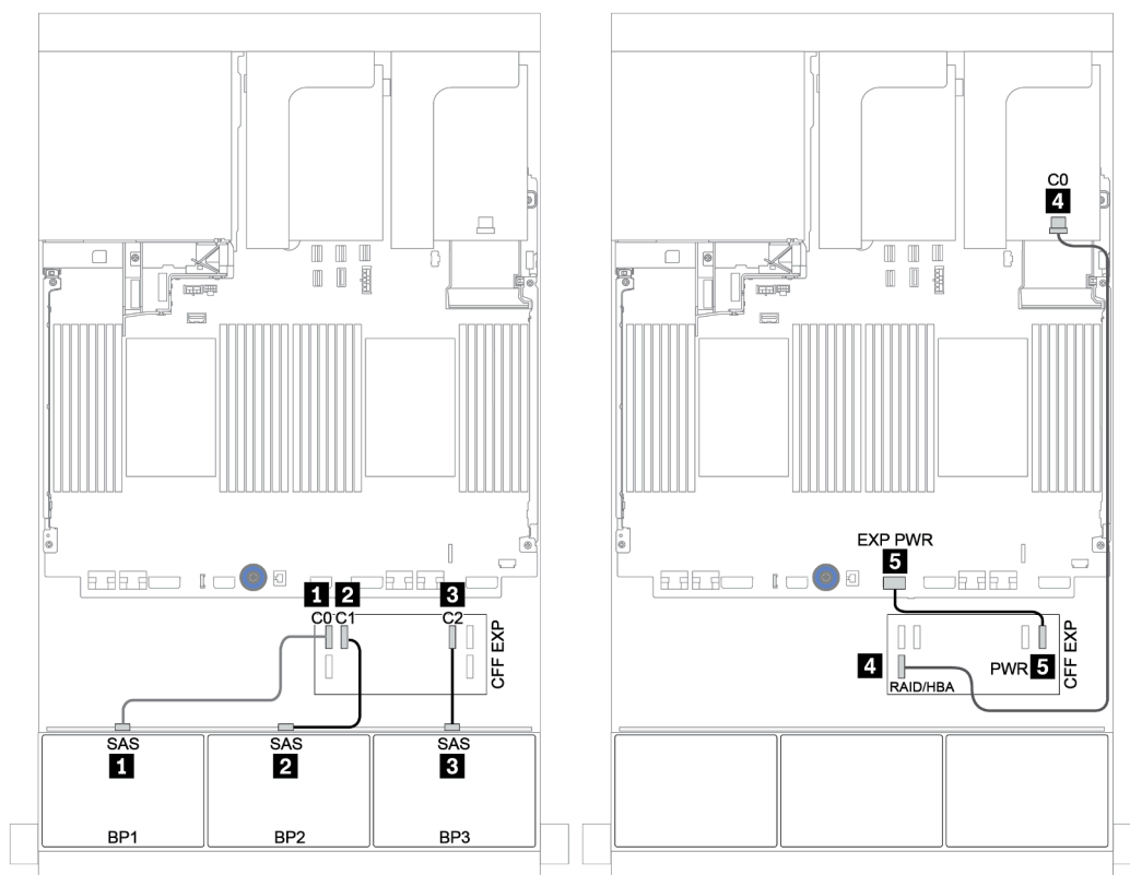
图 142. SAS/SATA 线缆布放
