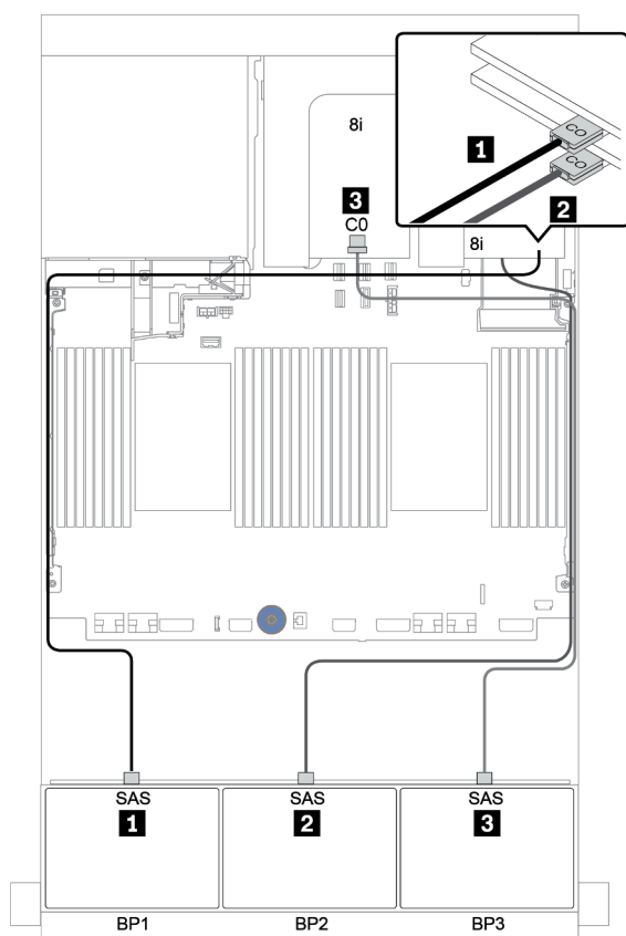
图 107. 配备一个 8i/16i RAID/HBA 适配器 和两个三模式 8i RAID 适配器 的 8 x 2.5 英寸 SAS/SATA + 16 x 2.5 英寸 AnyBay 配置的线缆布放
