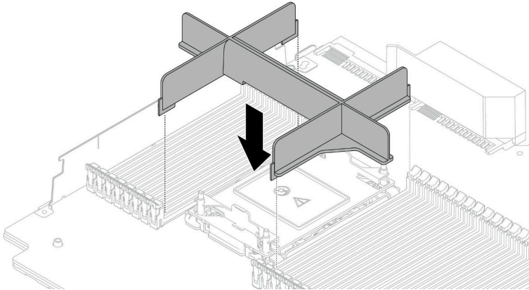
图 276. 安装 PHM 填充件
