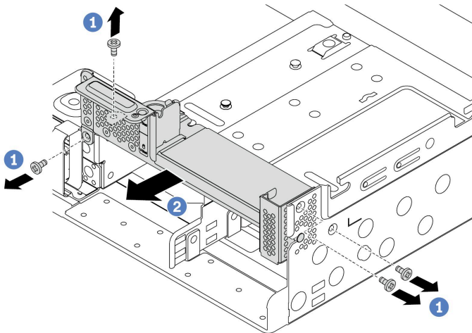
图 307. 卸下 C1 后壁支架（右侧）
