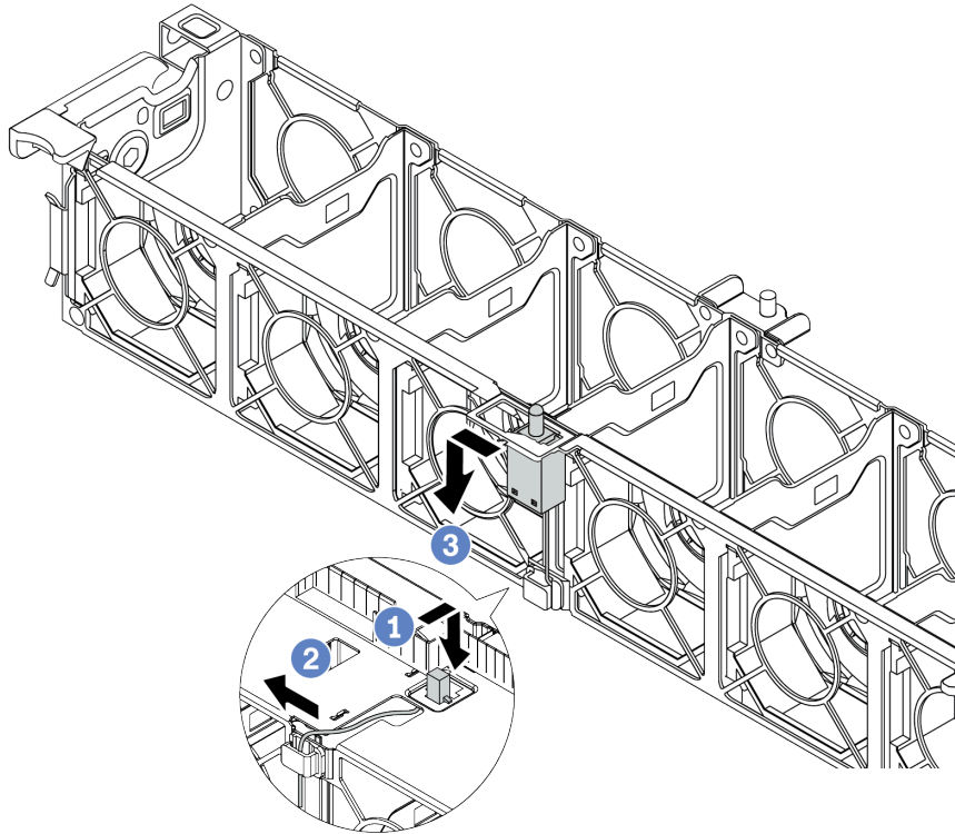
图 236. 卸下入侵感应开关
