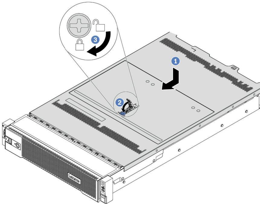
图 361. 安装顶盖
