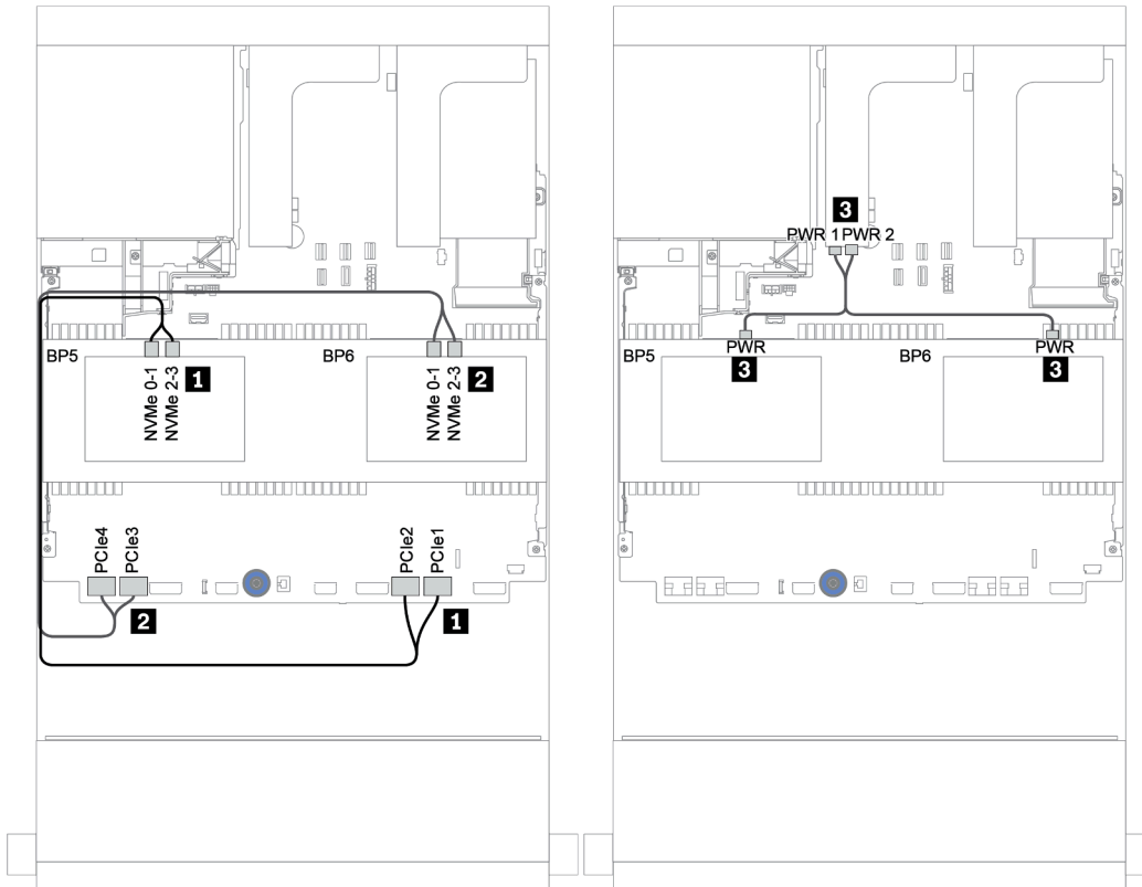
图 163. 两个 4 x 2.5 英寸 NVMe 中间硬盘背板的线缆布放
