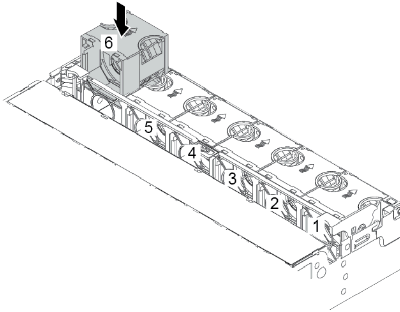
图 348. 安装系统风扇
