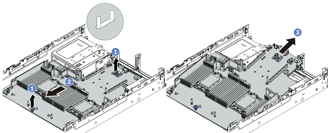
图 345. 卸下主板
