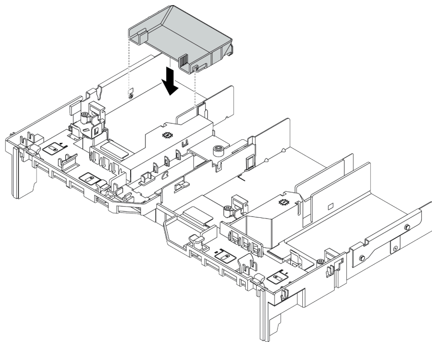
图 222. 安装附加导风罩
