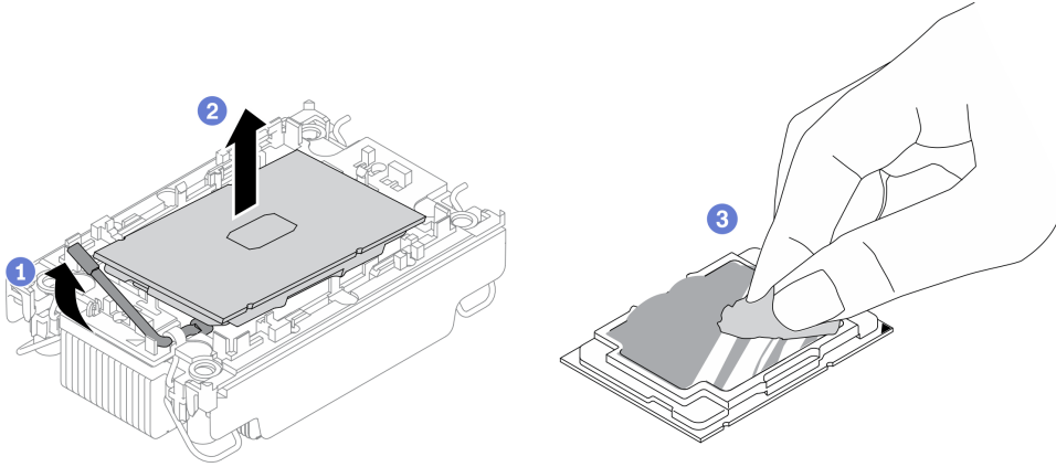
图 277. 将处理器与散热器和支架分开
