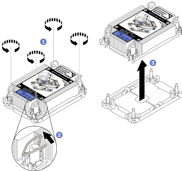
图 275. 卸下 PHM
