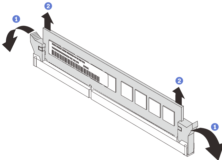
图 248. 卸下内存条
