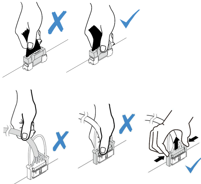
图 218. 从主板上拔下线缆
