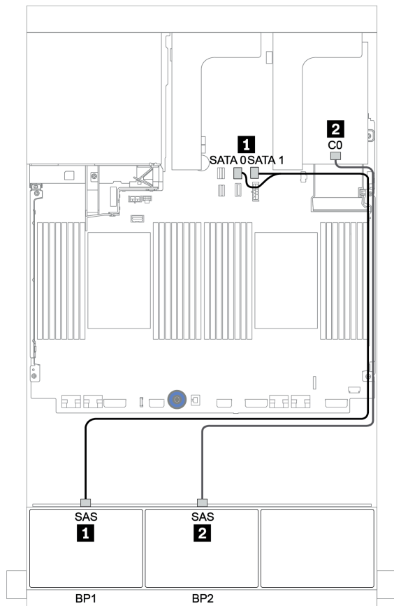
图 100. 配备一个三模式 8i RAID 适配器的 8 x 2.5 英寸 SAS/SATA + 8 x 2.5 英寸 AnyBay 配置的线缆布放
