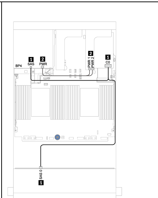
图 188. 配备 RAID 940-8i 适配器时的线缆布放
