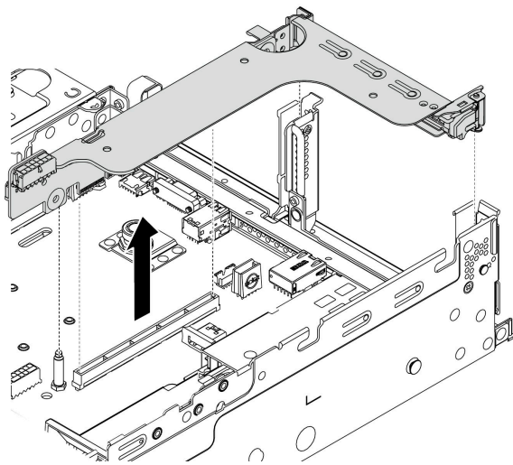
图 352. 卸下转接卡支架
