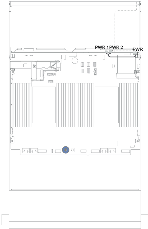
圖例 175. 後方背板的電源線佈線
