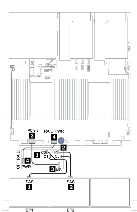
圖例 39. 配置為一個 CFF 16i RAID/HBA 配接卡的 16 x 2.5 吋 SAS/SATA 的纜線佈線
