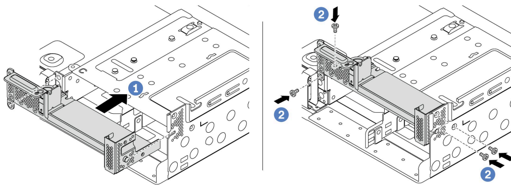
圖例 310. 安裝 C1 後壁托架 (右)
