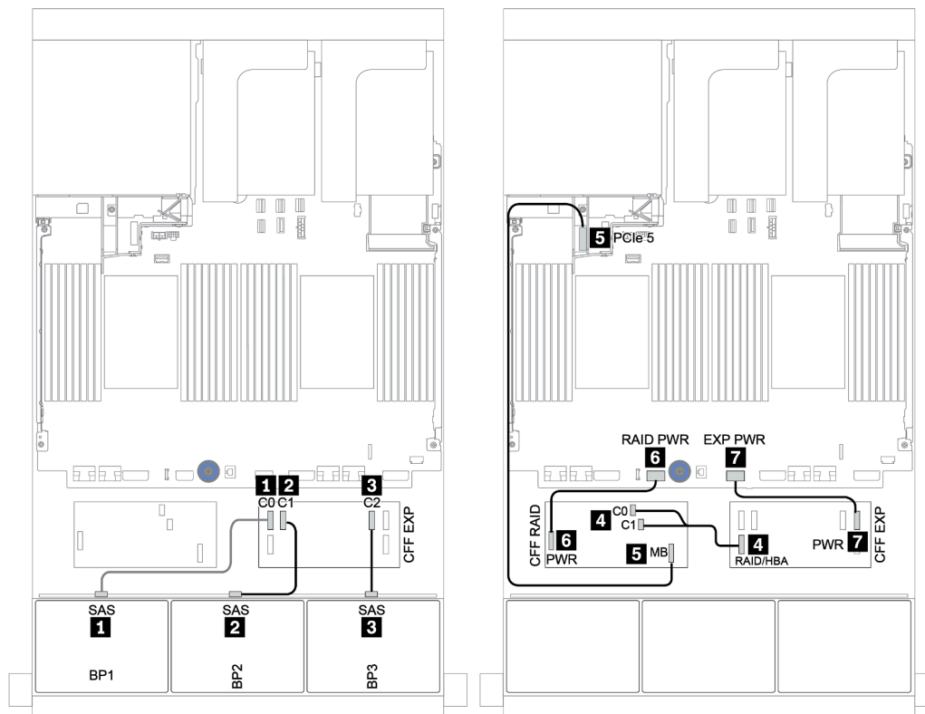
圖例 136. SAS/SATA 纜線佈線
