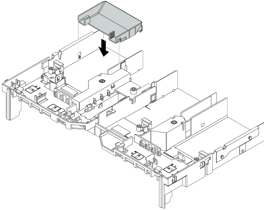
圖例 222. 安裝空氣擋板附加元件
