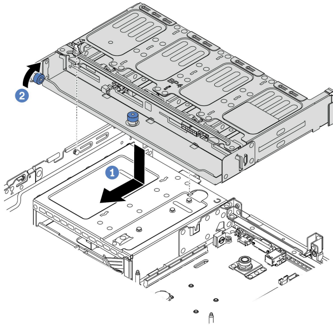
圖例 318. 安裝 8 x 2.5 吋背面框架
