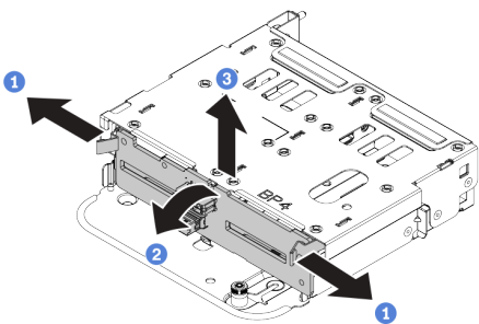
圖例 313. 卸下後方 4 x 2.5 吋硬碟背板
