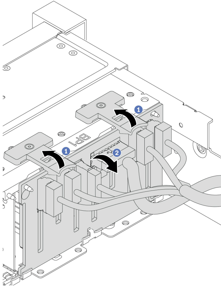
圖例 204. 卸下 2.5 吋硬碟背板
