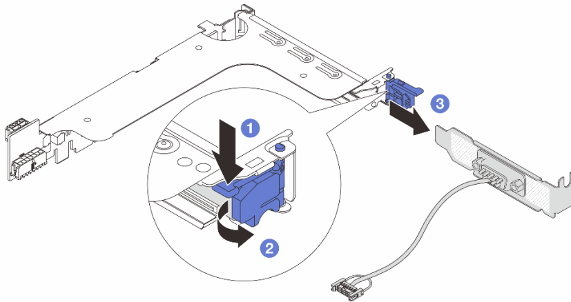
圖例 353. 卸下序列埠模組
