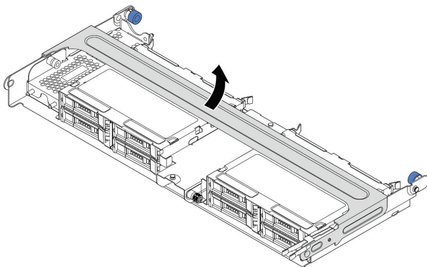
圖例 302. 打開中間框架的把手
