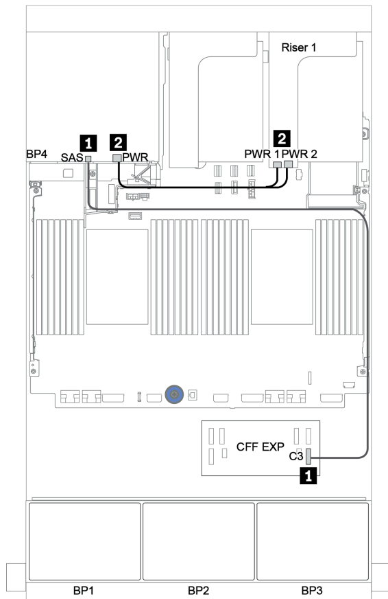
圖例 138. 後方 4 x 2.5 吋 SAS/SATA 背板的纜線佈線
