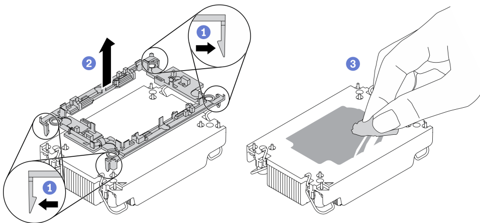
圖例 278. 將處理器支架與散熱槽分開
