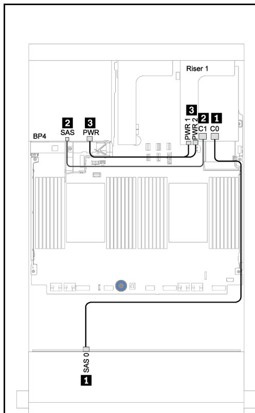
圖例 187. 包含 RAID 930/9350-8i 配接卡的纜線佈線
