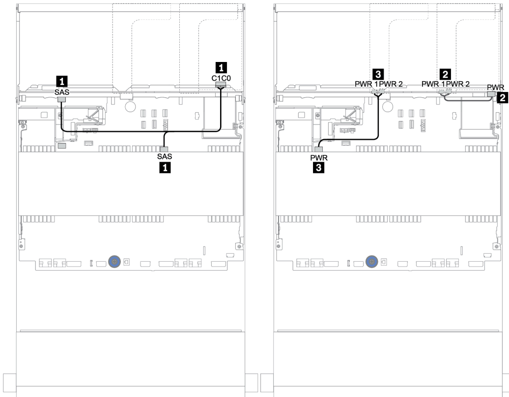
圖例 165. 4 x 3.5 吋 SAS/SATA 中間背板和 4 x 3.5 吋 SAS/SATA 後方背板的纜線佈線
