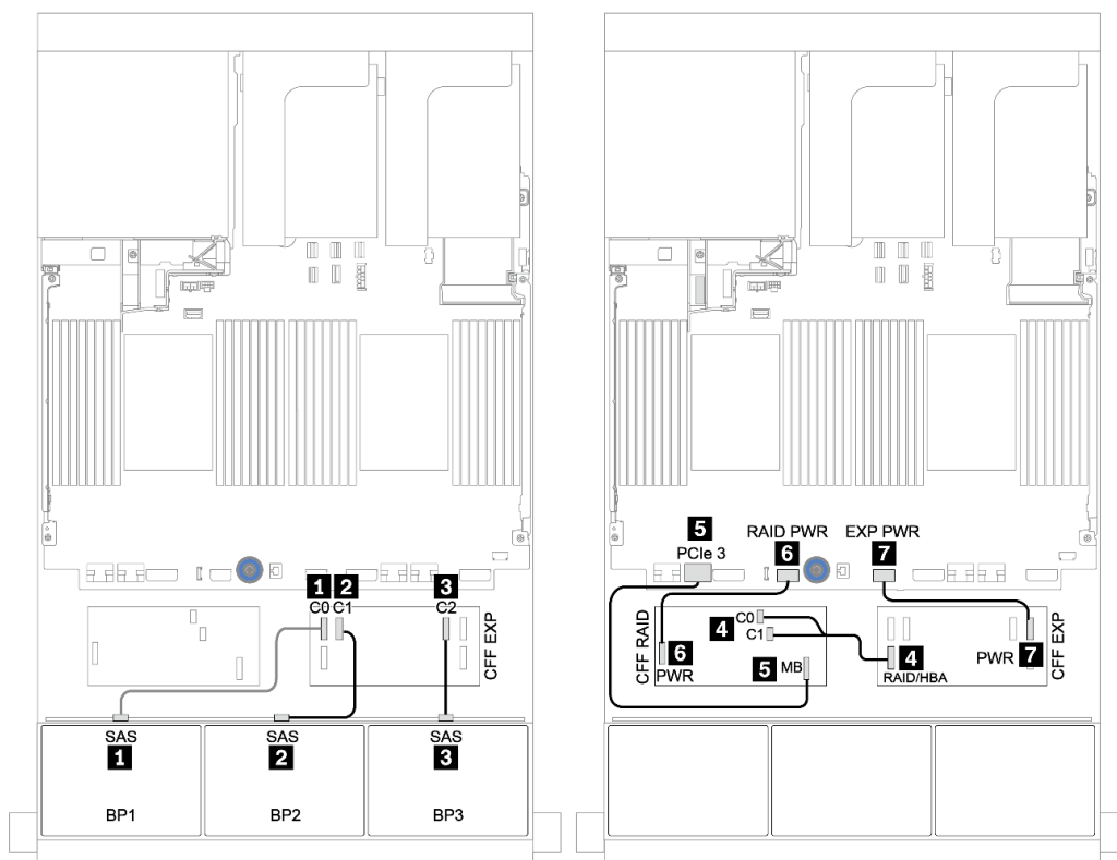
圖例 44. 配置為一個 CFF 16i RAID/HBA 配接卡和一個 CFF 擴充器的 24 x 2.5 吋 SAS/SATA 的纜線佈線
