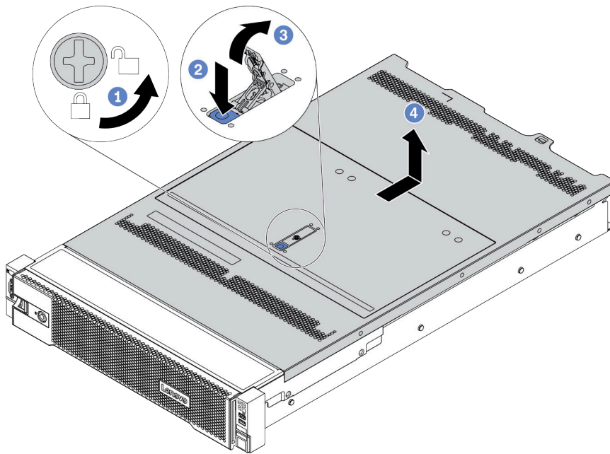
圖例 358. 卸下上蓋
