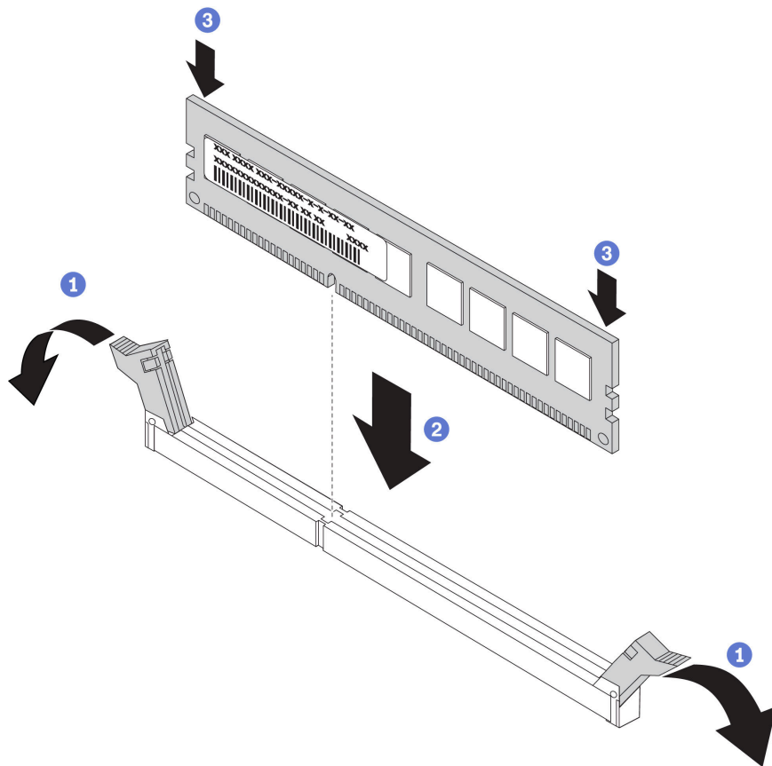
圖例 249. 安裝記憶體模組
