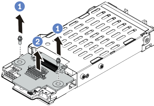
圖例 331. 卸下 7 公釐硬碟背板 (頂端)
