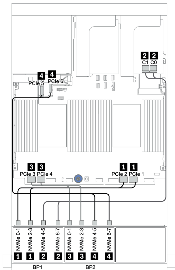
圖例 65. 配置為一個重定時器卡的 16 x 2.5 吋 NVMe 的纜線佈線
