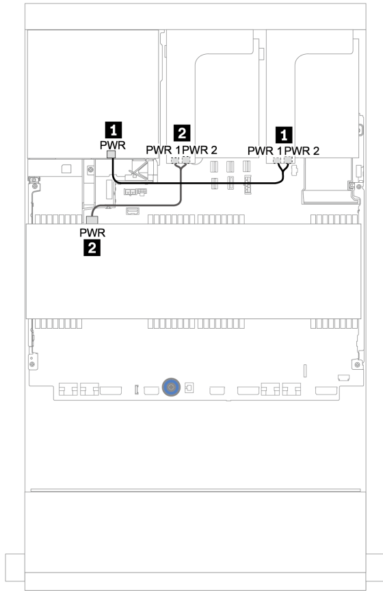
圖例 184. 中間和後方背板的電源線佈線
