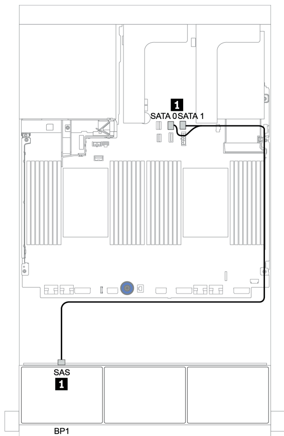
圖例 33. 配置為機載接頭的 8 x 2.5 吋 SAS/SATA 的纜線佈線
