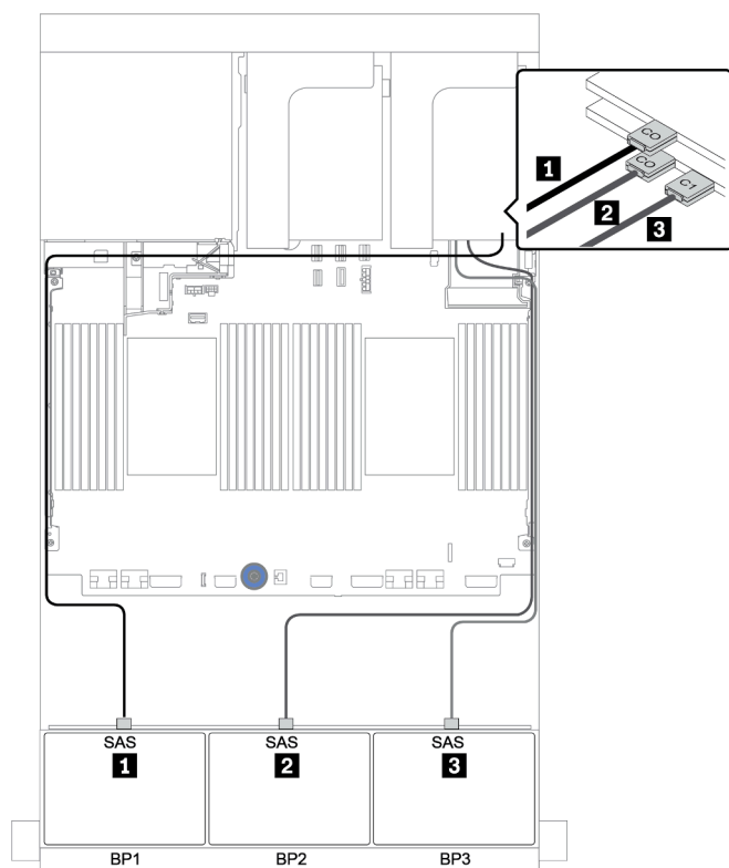
圖例 108. 配置為一個 8i/16i RAID/HBA 配接卡和一個三模式 16i RAID 配接卡的 8 x 2.5 吋 SAS/SATA + 16 x 2.5 吋 AnyBay 的纜線佈線
