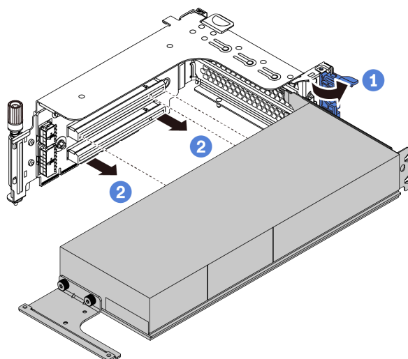
圖例 220. 卸下 GPU 配接卡
