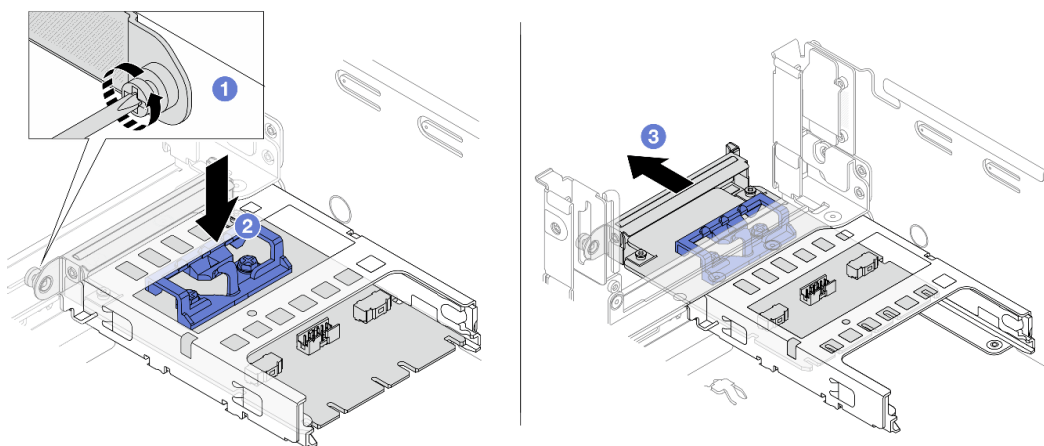
圖例 338. 卸下 vSphere DSE 的 OCP 啟用套件
