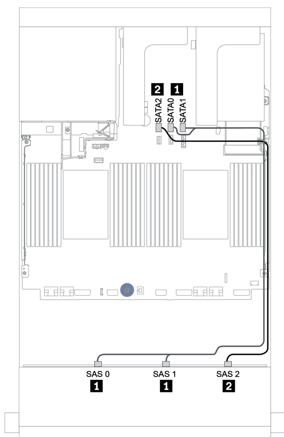
圖例 164. 配備機載接頭的 12 x 3.5 吋 SAS/SATA 前方背板的纜線佈線
