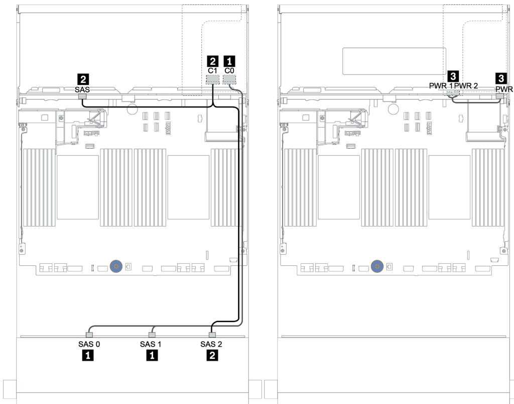
圖例 155. 配置為 4 x 3.5 吋 SAS/SATA 後方背板的 12 x 3.5 吋 SAS/SATA 的纜線佈線
