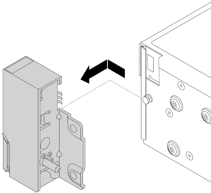
圖例 288. 機架門鎖拆卸
