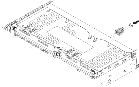
圖例 327. 安裝上蓋支撐托架
