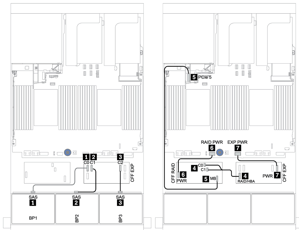
圖例 121. SAS/SATA 纜線佈線
