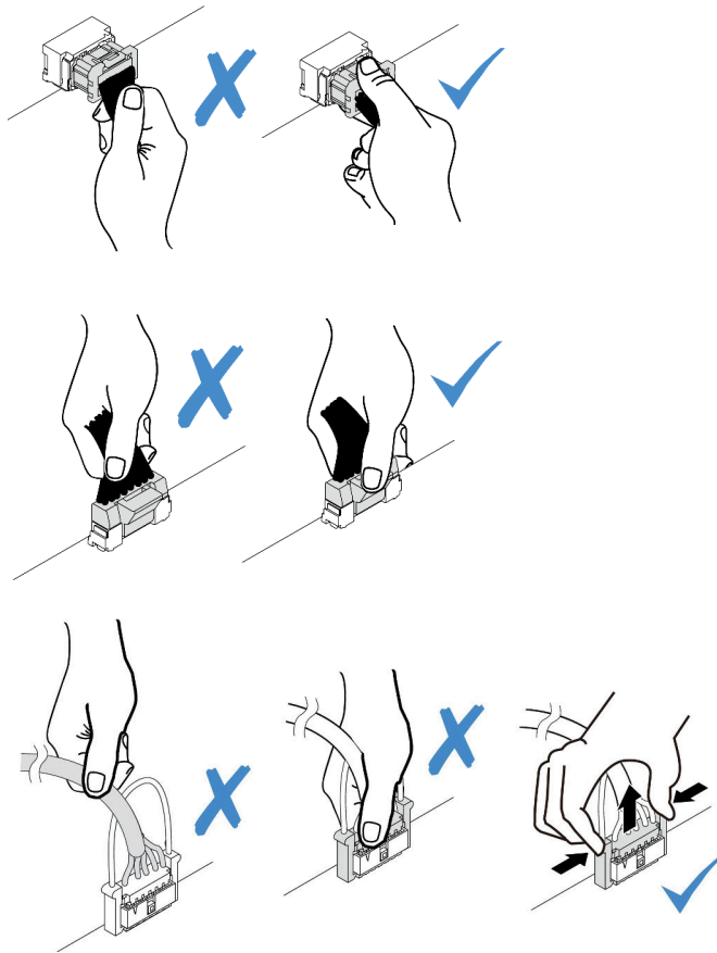
圖例 285. 從主機板拔掉纜線
