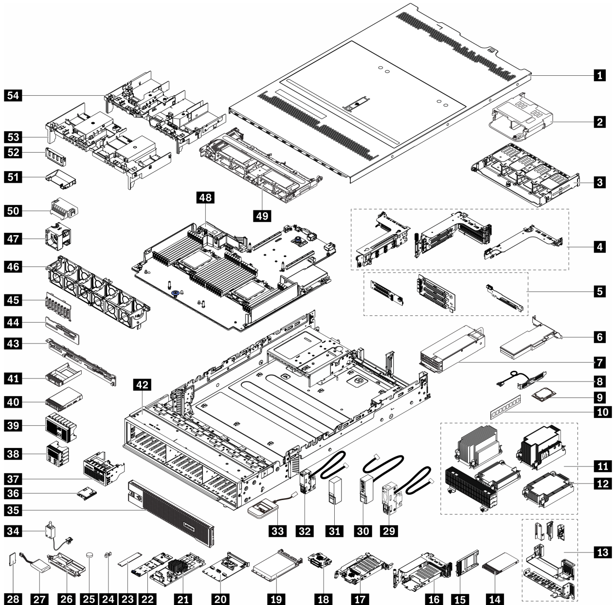
圖例 14. 伺服器元件 (2.5 吋機槽機箱)
