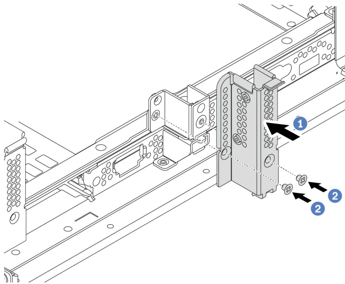
圖例 309. 安裝 B1 後壁托架 (中間)
