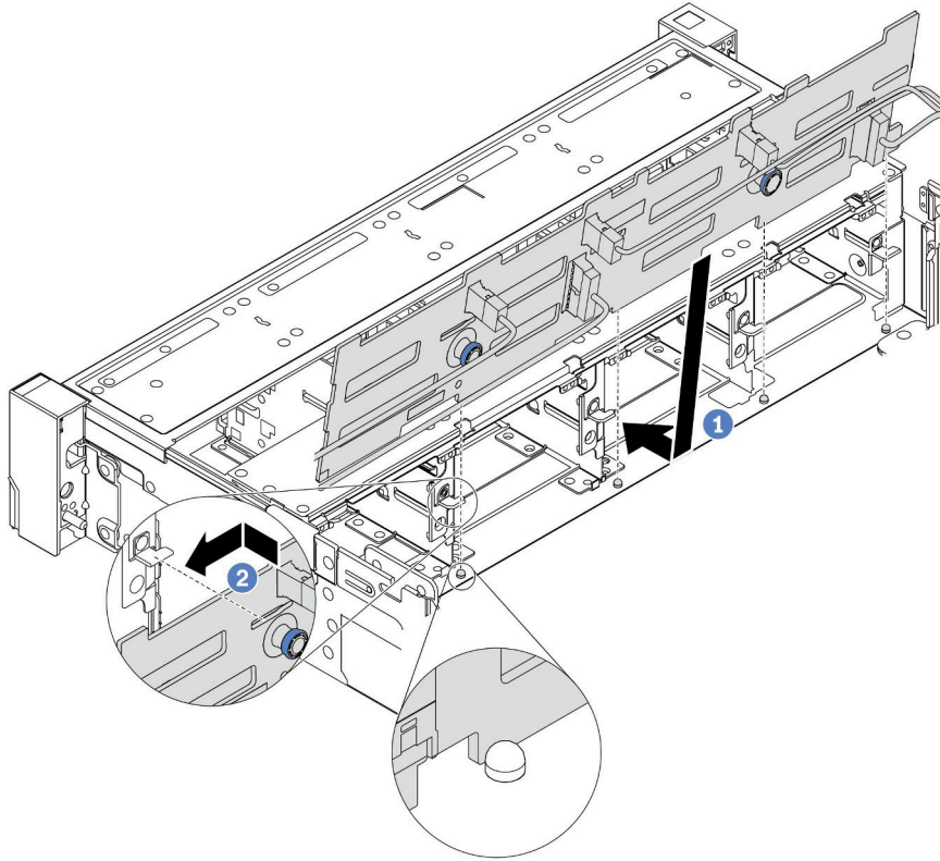
圖例 208. 安裝 3.5 吋硬碟背板
