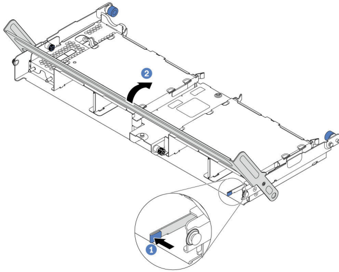
圖例 251. 關上框架把手
