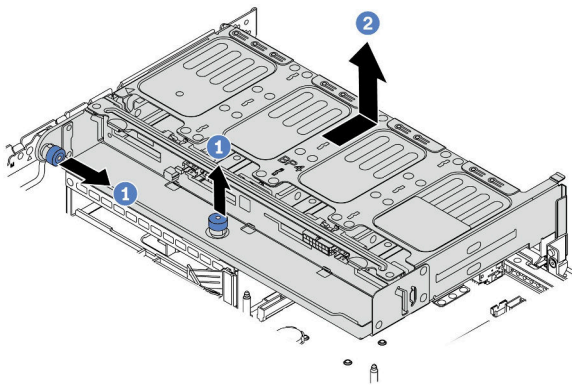
圖例 312. 卸下 8 x 2.5 吋背面框架
