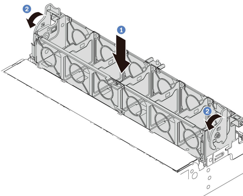
圖例 350. 系統風扇機盒安裝
