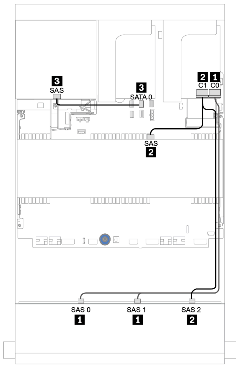
圖例 167. SAS/SATA 纜線佈線
