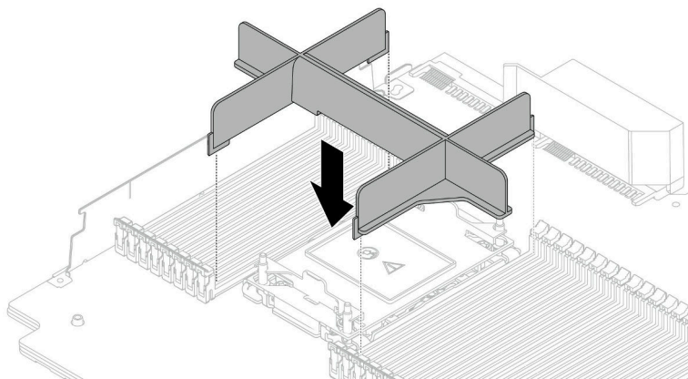
圖例 276. 安裝 PHM 填充板
