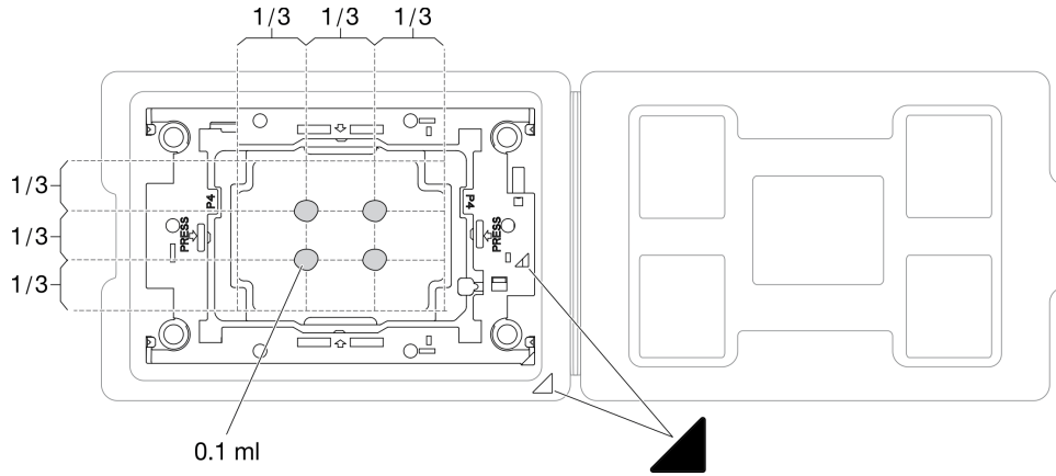
圖例 281. 運送匣中的處理器塗上散熱膏
