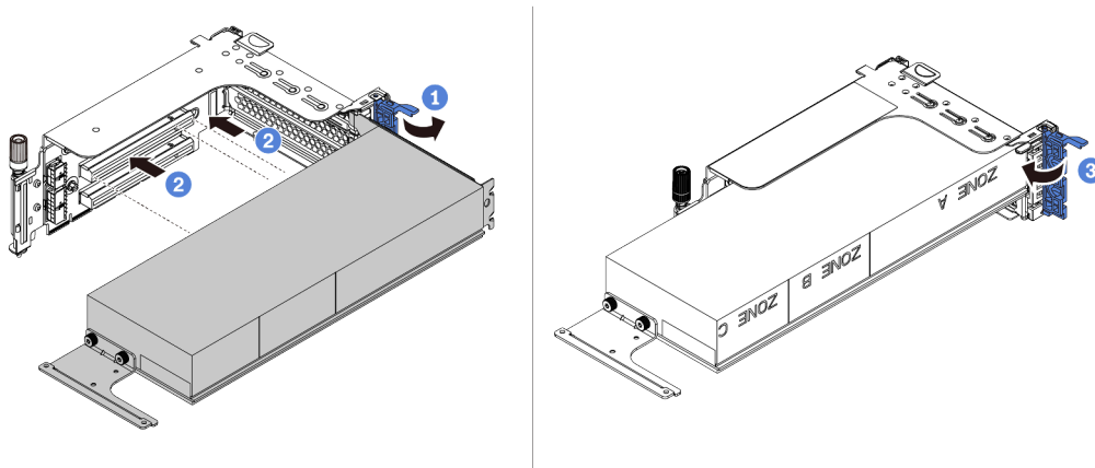
圖例 221. 安裝 GPU 配接卡
