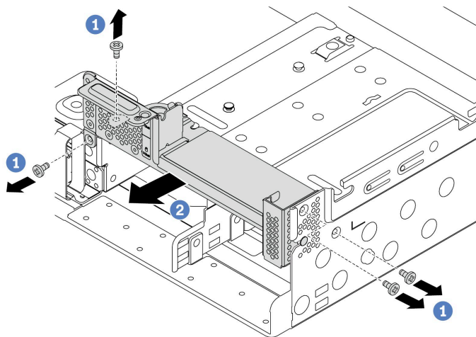
圖例 307. 卸下 C1 後壁托架 (右)
