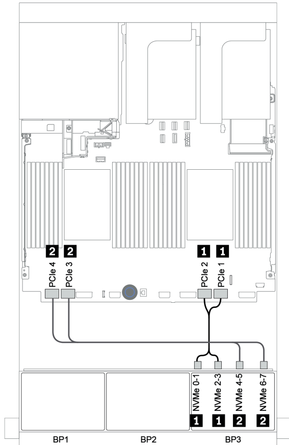
圖例 134. NVMe 纜線佈線 (兩個處理器)
