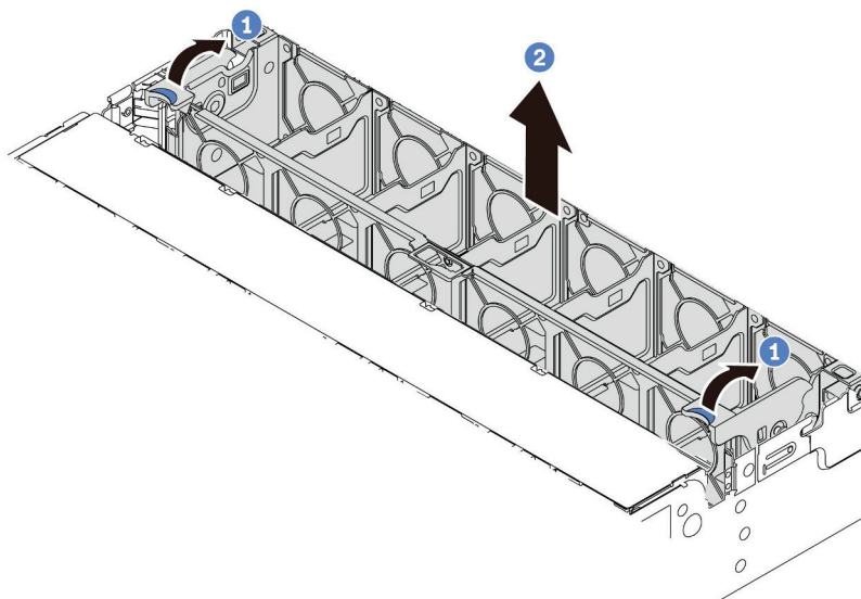
圖例 349. 卸下系統風扇機盒
