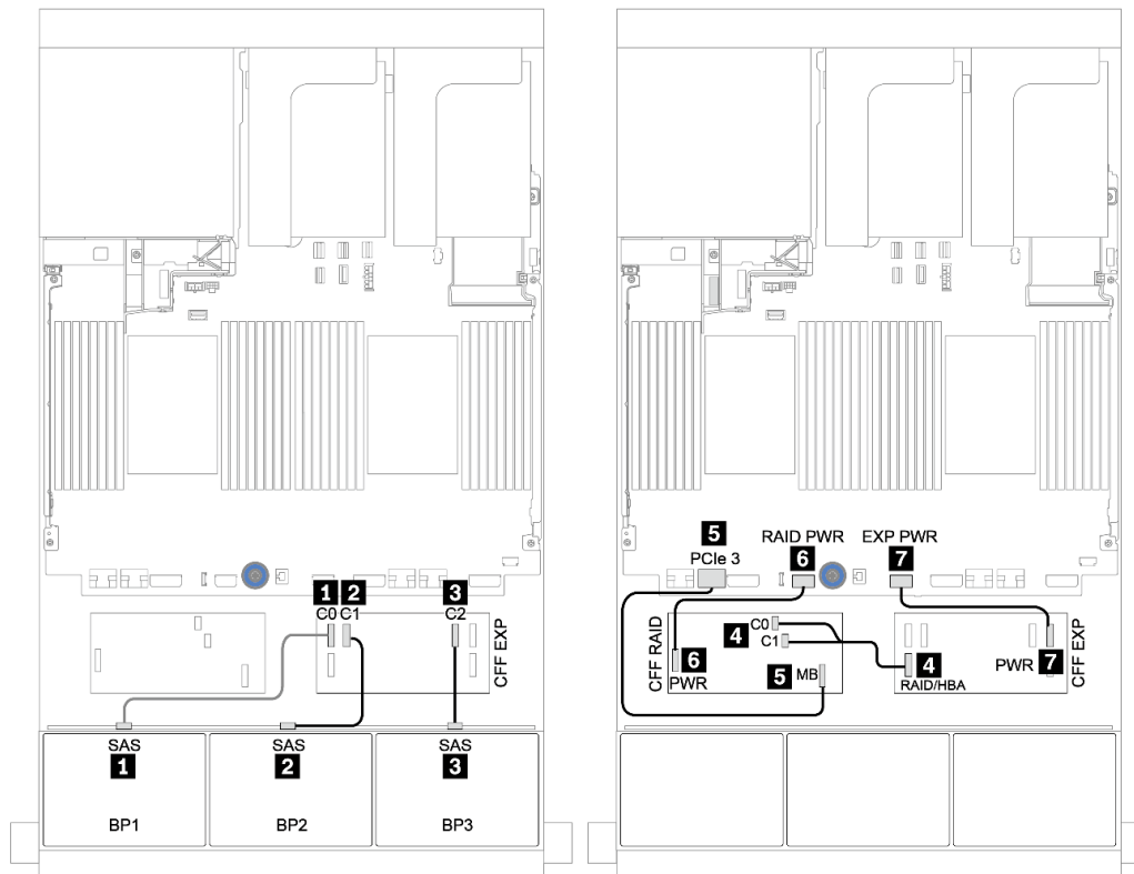
圖例 57. 配置為一個 CFF 16i RAID/HBA 配接卡和一個 CFF 擴充器的 24 x 2.5 吋 SAS/SATA 的纜線佈線
