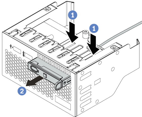
圖例 213. 卸下整合式診斷面板
