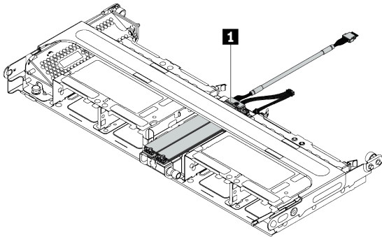
圖例 28. 在 8 x 2.5 中間框架上
