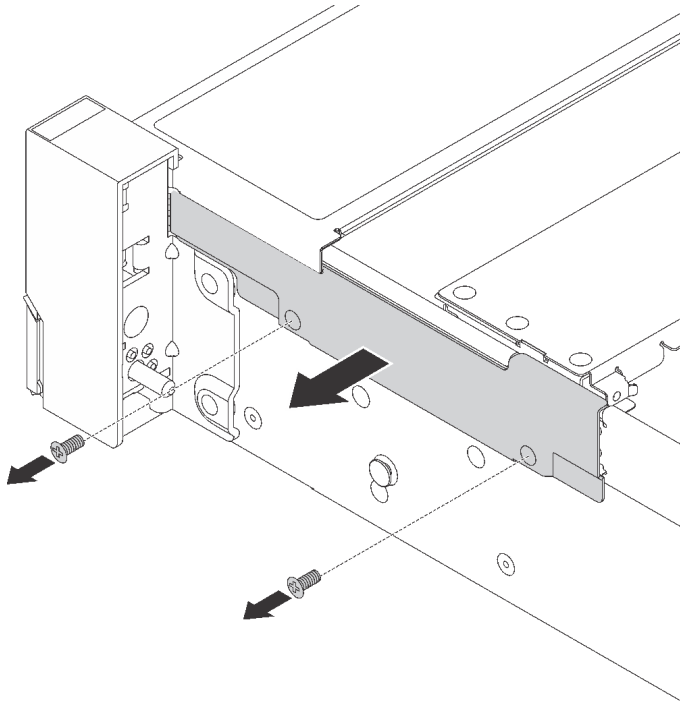
圖例 286. 卸下纜線固定夾
