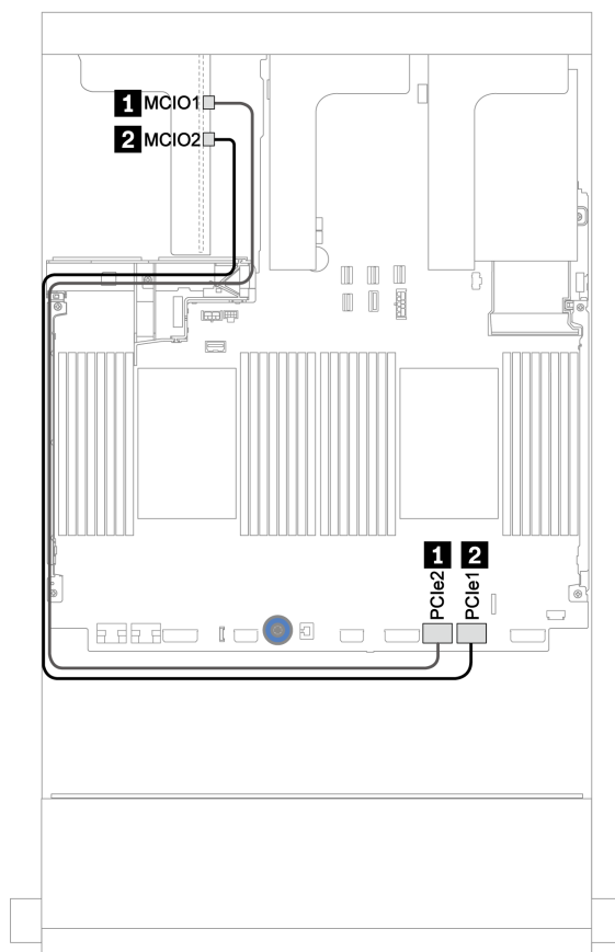
圖例 19. x8/x8 PCIe 擴充卡 3 的纜線佈線 ( 一個處理器 )
