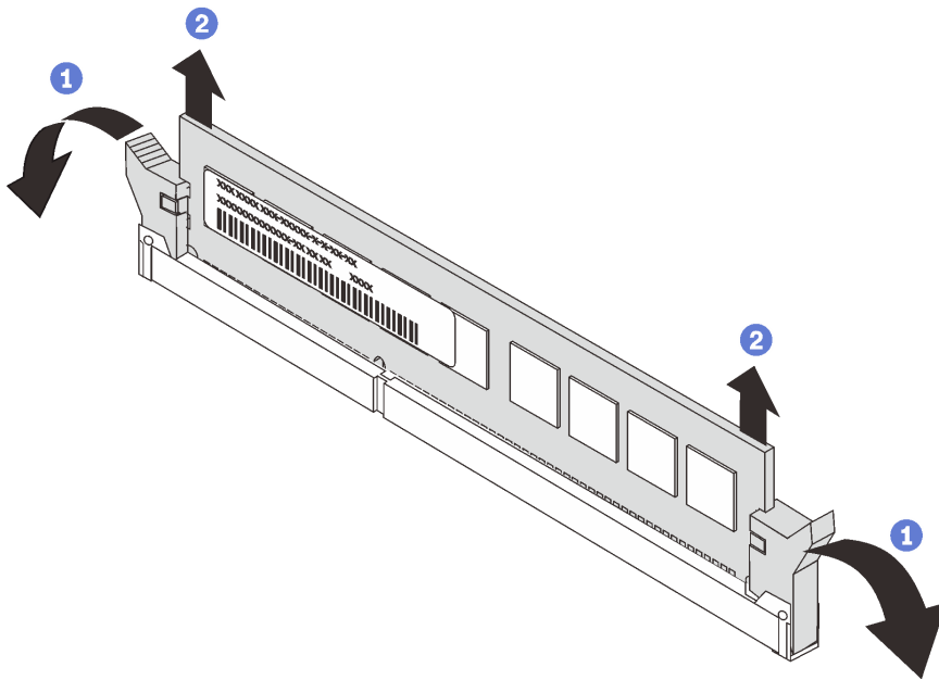
圖例 248. 卸下記憶體模組
