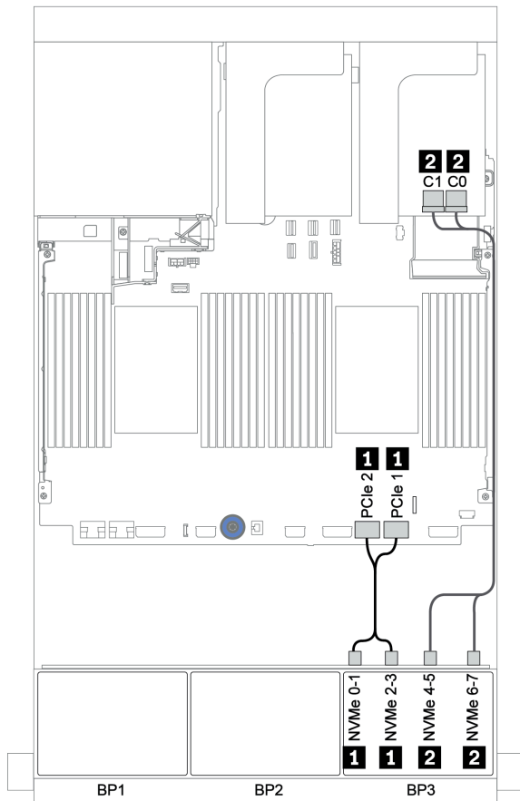
圖例 126. NVMe 纜線佈線 (一個處理器)
