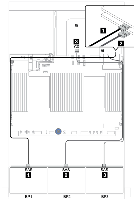
圖例 115. SAS/SATA 纜線佈線
