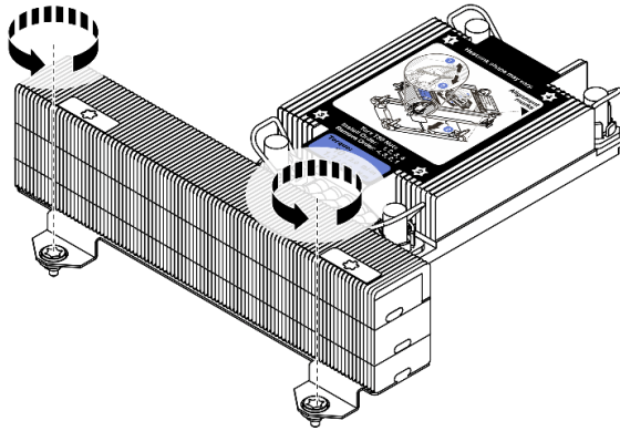
圖例 274. 鬆開 T 形散熱槽螺絲
