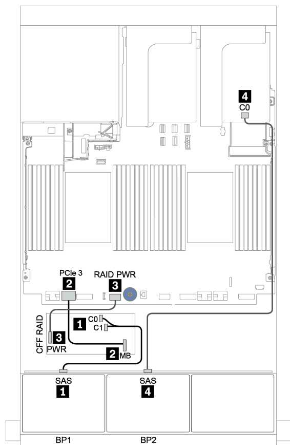
圖例 102. 配置為一個 CFF 16i RAID/HBA 配接卡和一個三模式 8i RAID 配接卡的 8 x 2.5 吋 SAS/SATA + 8 x 2.5 吋 AnyBay 的纜線佈線
