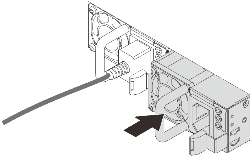
圖例 272. 安裝熱抽換電源供應器
