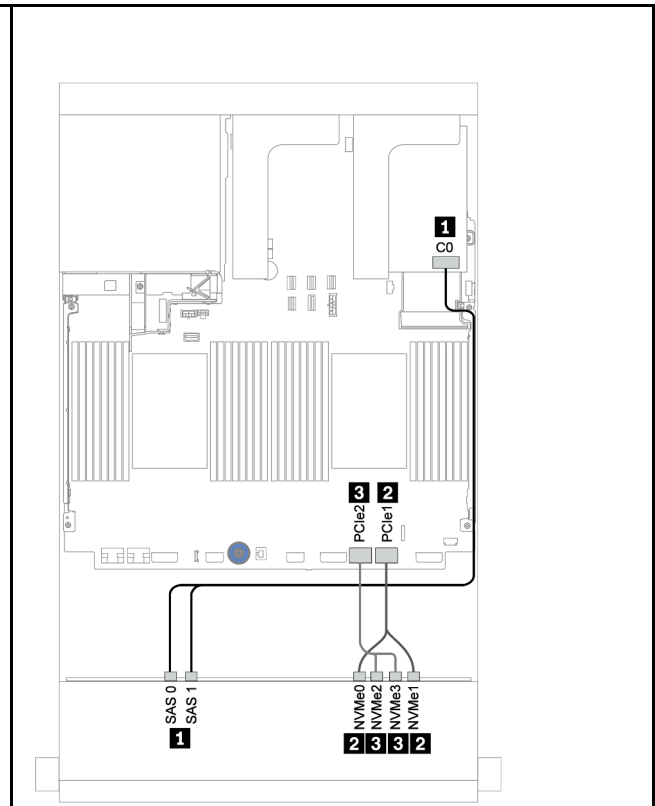
圖例 190. 包含 RAID 940-8i 配接卡的纜線佈線
