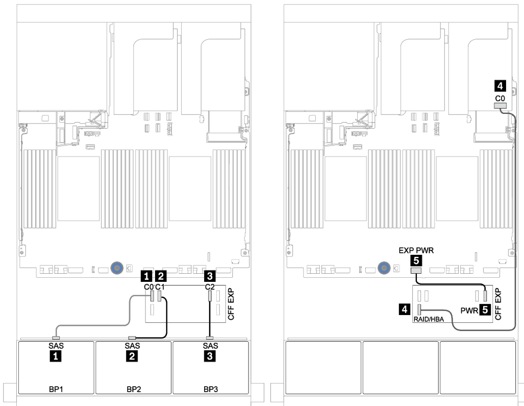
圖例 53. 配置為一個 8i 配接卡和一個 CFE 擴充器的 24 x 2.5 吋 SAS/SATA 的纜線佈線
