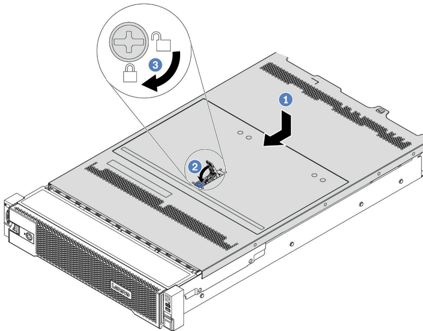
圖例 361. 安裝上蓋
