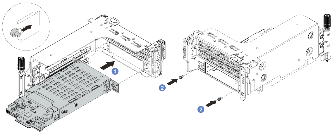
圖例 336. 安裝 7 公釐框架
