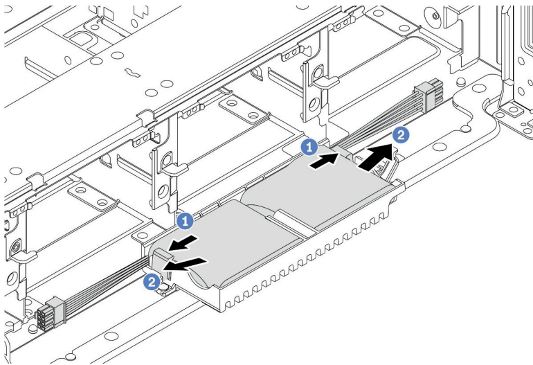
圖例 296. 卸下 RAID 快閃記憶體電源模組
