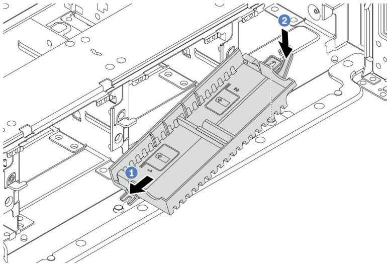
圖例 298. 安裝超級電容固定器
