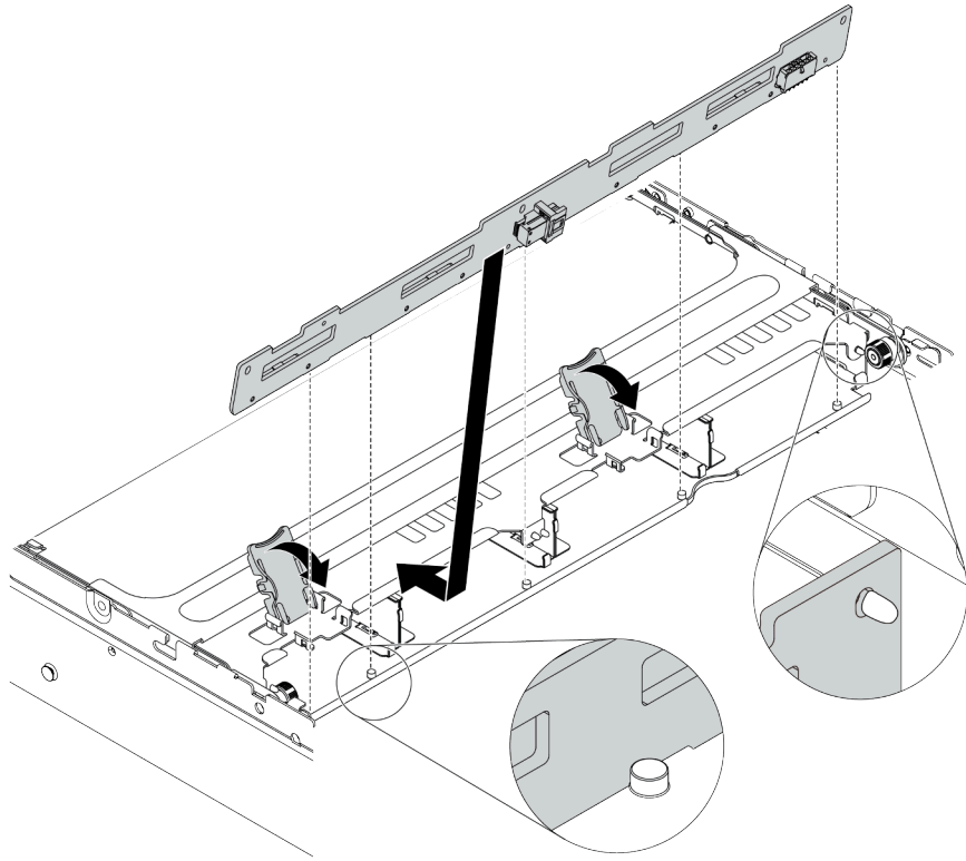
圖例 255. 安裝 3.5 吋中間硬碟背板
