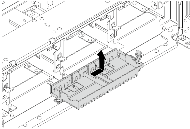
圖例 297. 卸下超級電容固定器
