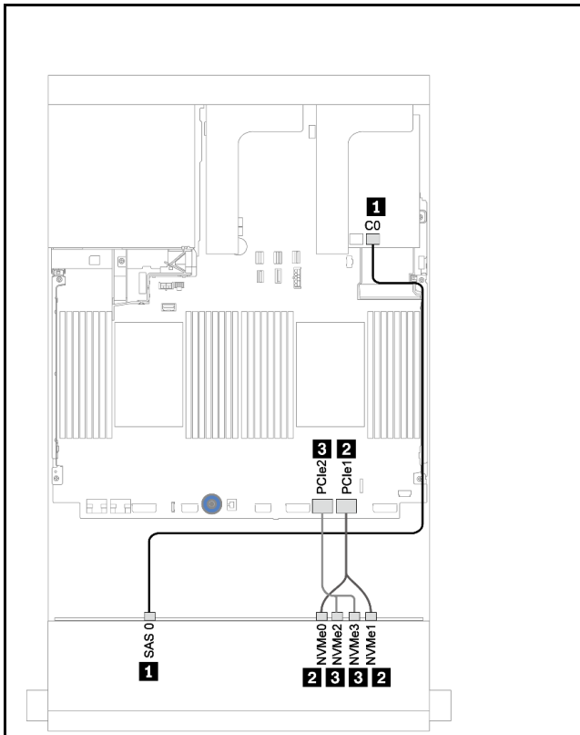
圖例 189. 包含 RAID 930/9350-8i 配接卡的纜線佈線
