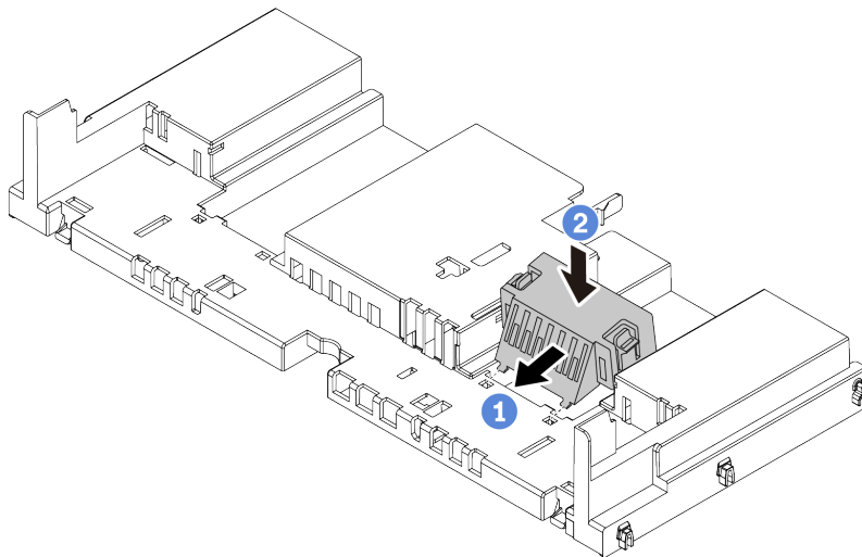
圖例 198. 空氣擋板填充板安裝
