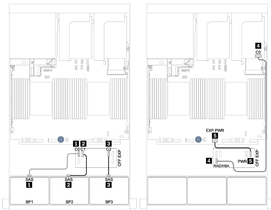
圖例 61. 配置為一個 CFF 擴充器和一個 430/4350-16i 配接卡的 24 x 2.5 吋 SAS/SATA 的纜線佈線
