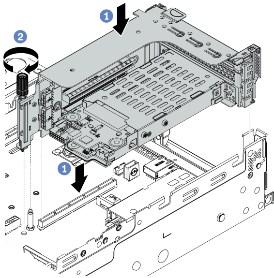
圖例 337. 安裝擴充卡組件
