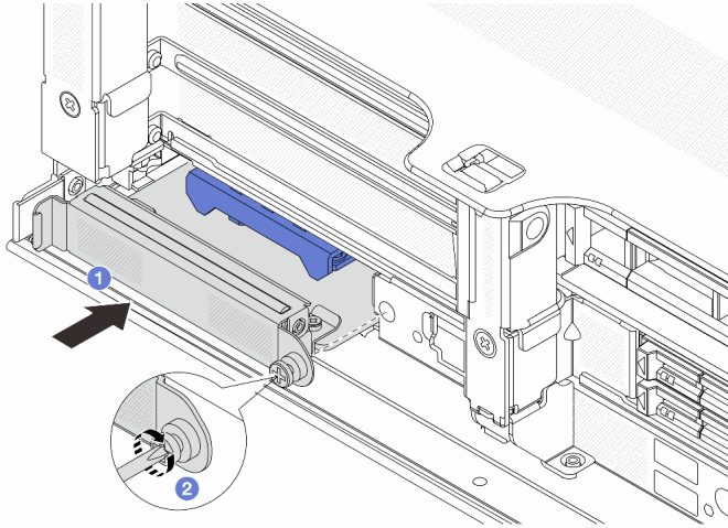
圖例 339. 安裝 vSphere DSE 的 OCP 啟用套件
