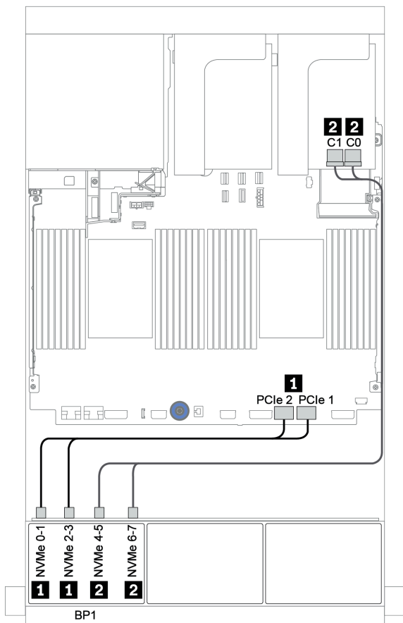
圖例 64. 配置為一個重定時器卡的 8 x 2.5 吋 NVMe 的纜線佈線
