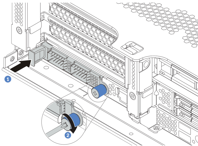
圖例 258. OCP 3.0 乙太網路配接卡安裝
