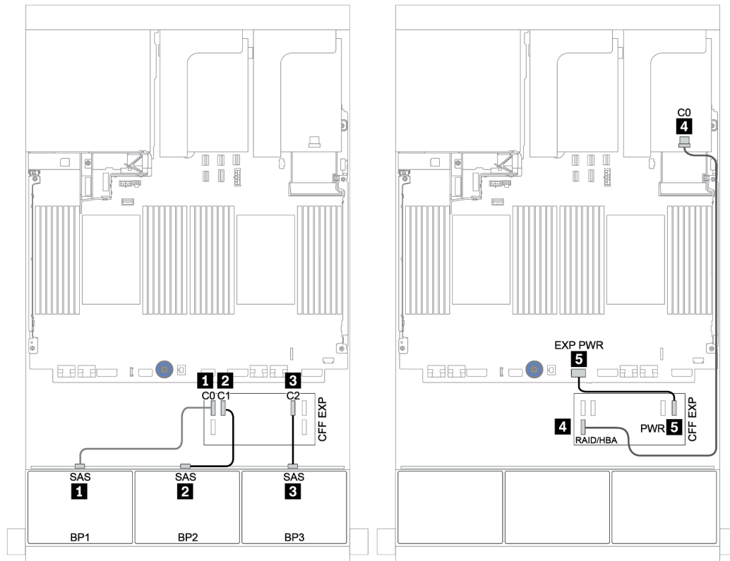
圖例 43. 配置為一個 CFF 擴充器和一個 8i RAID/HBA 配接卡的 24 x 2.5 吋 SAS/SATA 的纜線佈線
