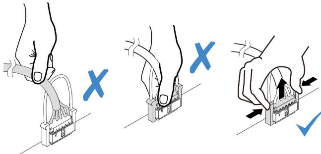
圖例 351. 拔掉序列埠纜線
