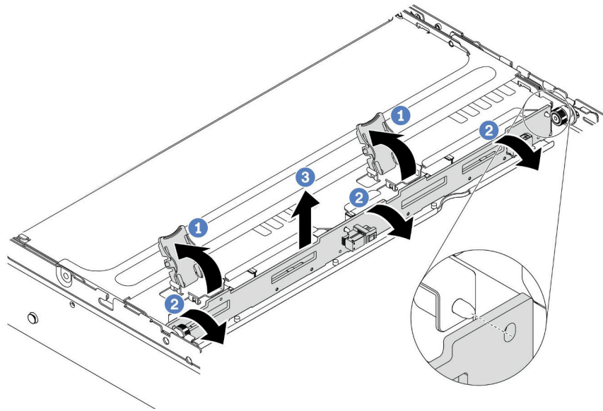
圖例 253. 卸下 3.5 吋中間硬碟背板
