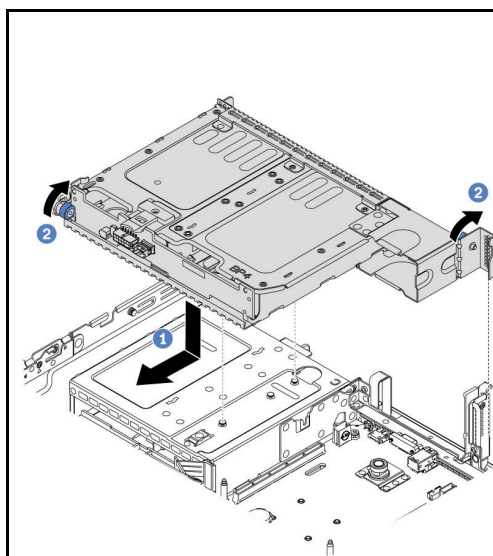
圖例 325. 安裝 2 x 3.5 吋背面框架
