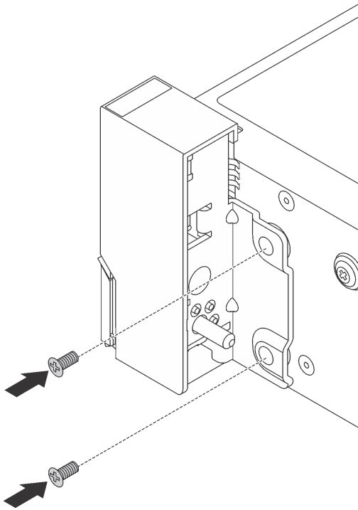
圖例 290. 螺絲安裝
