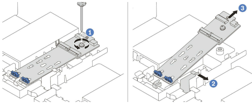
圖例 242. 卸下 M.2 背板
