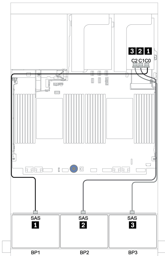
圖例 47. 配置為一個 32i RAID 配接卡的 24 x 2.5 吋 SAS/SATA 的纜線佈線
