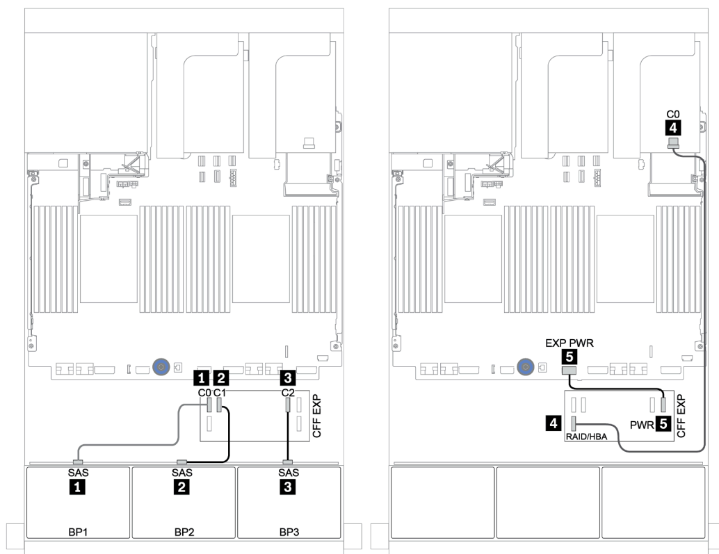
圖例 125. SAS/SATA 纜線佈線
