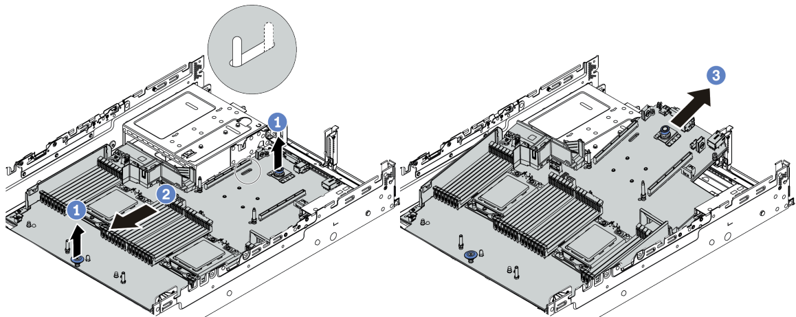
圖例 345. 卸下主機板
