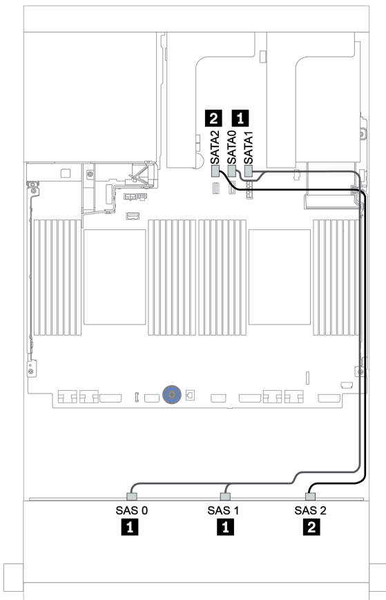
圖例 160. 配備機載接頭的 12 x 3.5 吋 SAS/SATA 前方背板的纜線佈線
