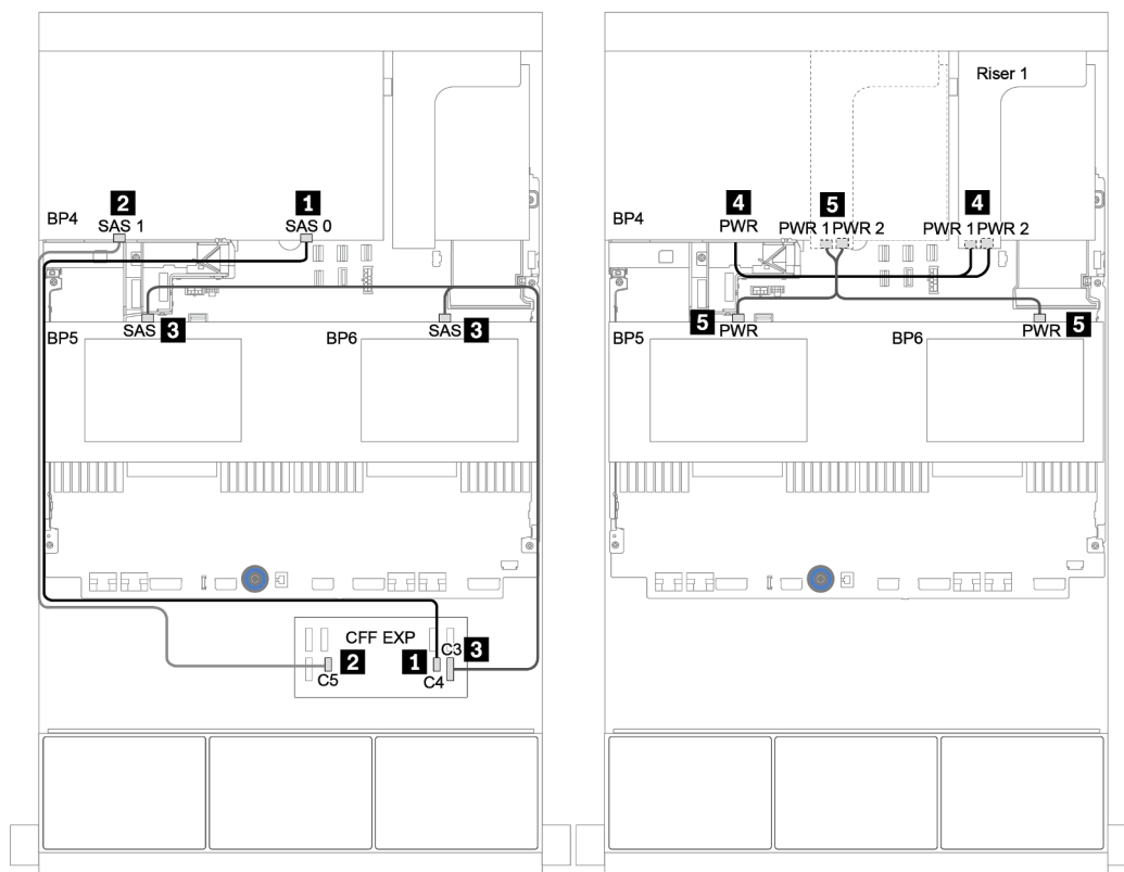
圖例 62. 中間 4 x 2.5 吋 SAS/SATA 背板和後方 8 x 2.5 吋 SAS/SATA 背板的纜線佈線
