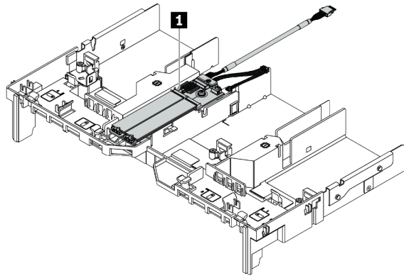
圖例 27. 在 GPU 空氣擋板上
