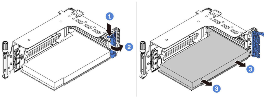
圖例 263. PCIe 配接卡拆卸
