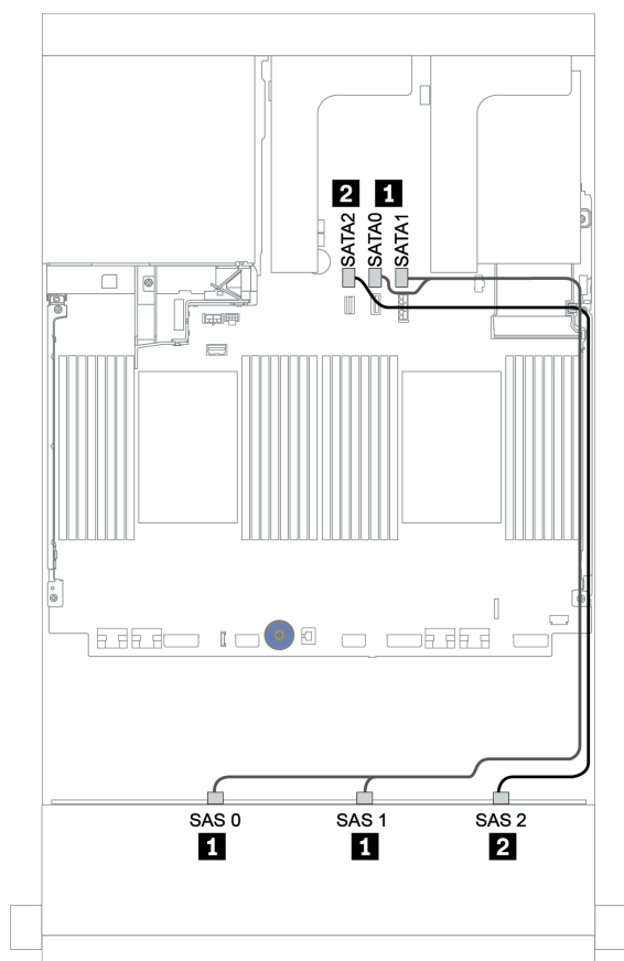
圖例 149. 配置為機載接頭的 12 x 3.5 吋 SAS/SATA 的纜線佈線
