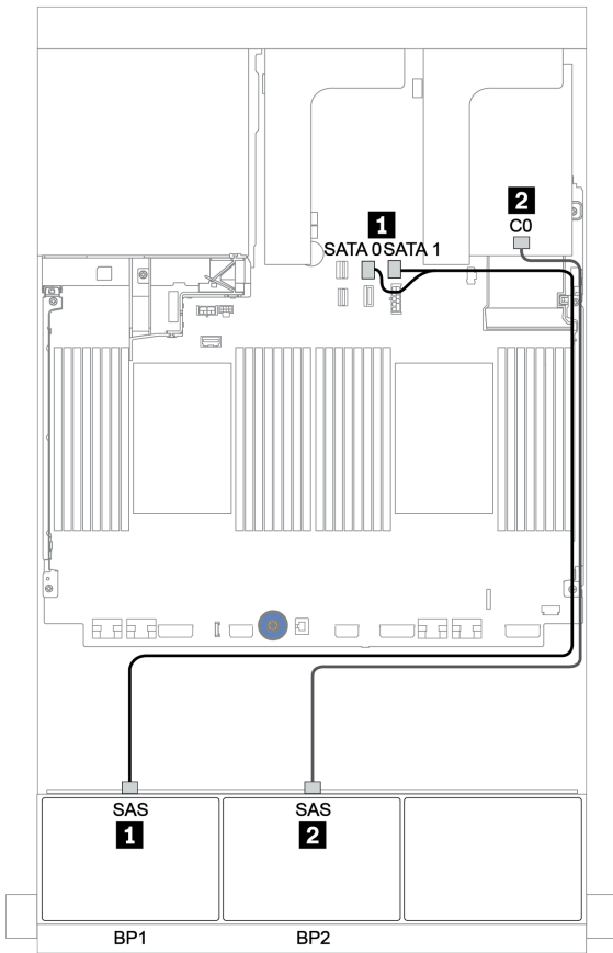
圖例 37. 配置為一個 8i RAID 配接卡的 16 x 2.5 吋 SAS/SATA 的纜線佈線
