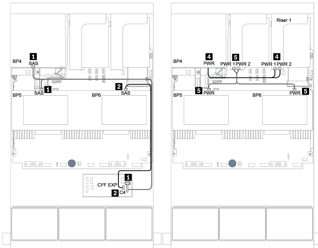
圖例 58. 4 x 2.5 吋 SAS/SATA 中間背板和 4 x 2.5 吋 SAS/SATA 後方背板的纜線佈線
