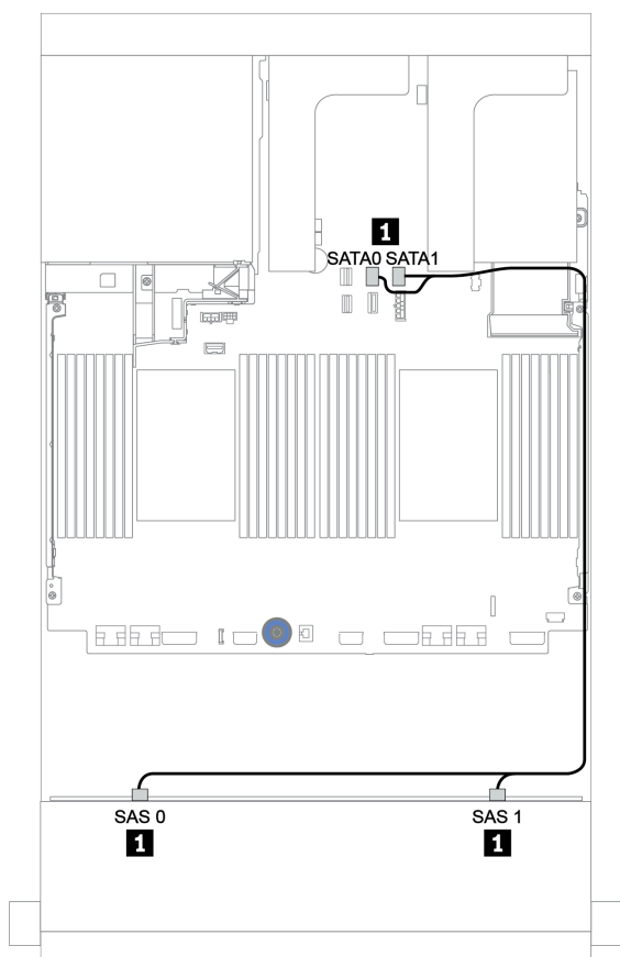
圖例 147. 配置為機載接頭的 8 x 3.5 吋 SAS/SATA 的纜線佈線
