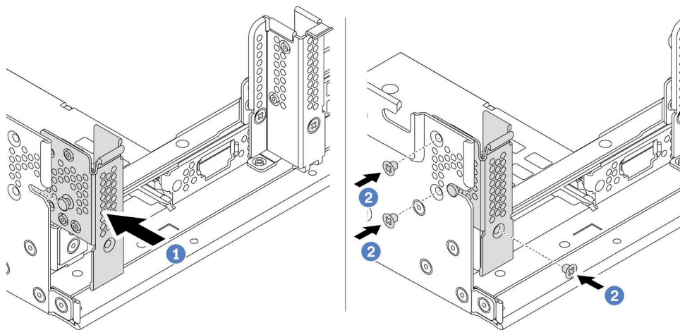
圖例 308. 安裝 A1 後壁托架 (左)
