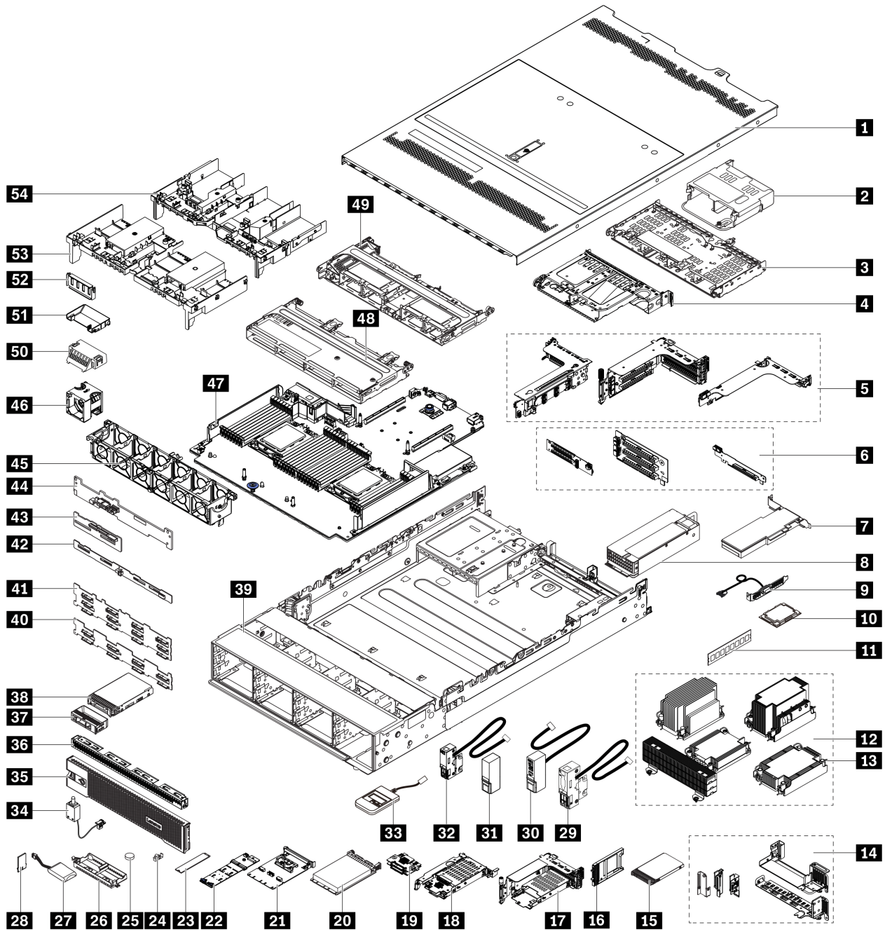
圖例 15. 伺服器元件 ( 3.5 吋機槽機箱 )
