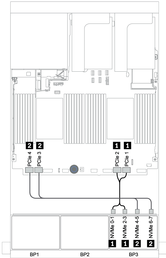
圖例 137. NVMe 纜線佈線
