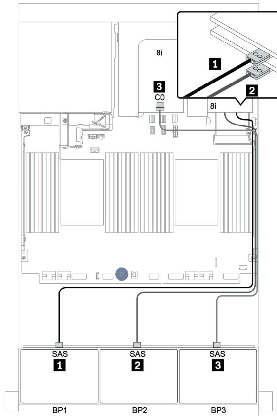
圖例 45. 配置為三個 8i RAID/HBA 配接卡的 24 x 2.5 吋 SAS/SATA 的纜線佈線
