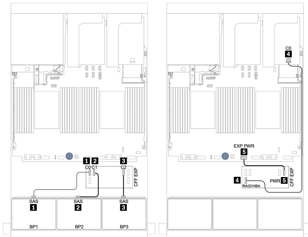
圖例 119. SAS/SATA 纜線佈線
