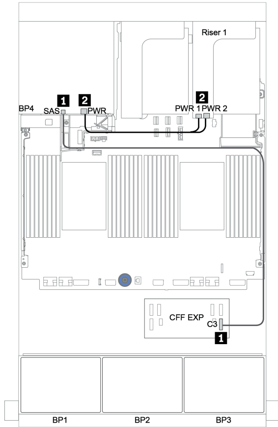
圖例 50. 4 x 2.5 吋 SAS/SATA 後方背板的纜線佈線
