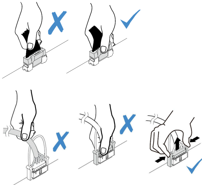
圖例 218. 從主機板拔掉纜線
