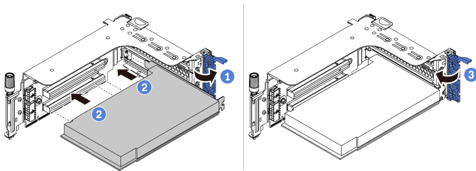
圖例 266. PCIe 配接卡安裝
