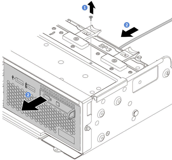
圖例 212. 卸下正面 I/O 模組
