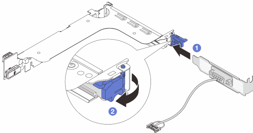
圖例 356. 安裝序列埠模組
