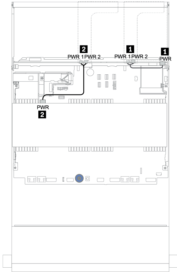
圖例 181. 中間和後方背板的電源線佈線
