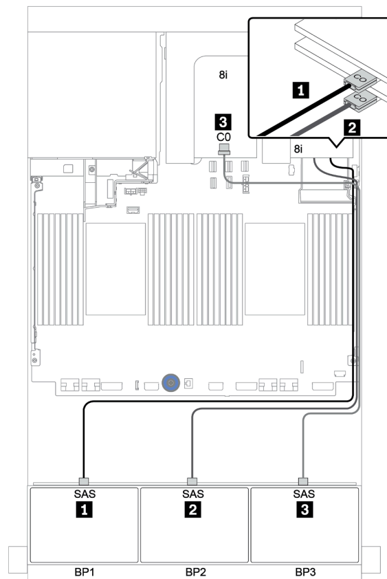
圖例 40. 配置為三個 8i RAID/HBA 配接卡的 24 x 2.5 吋 SAS/SATA 的纜線佈線
