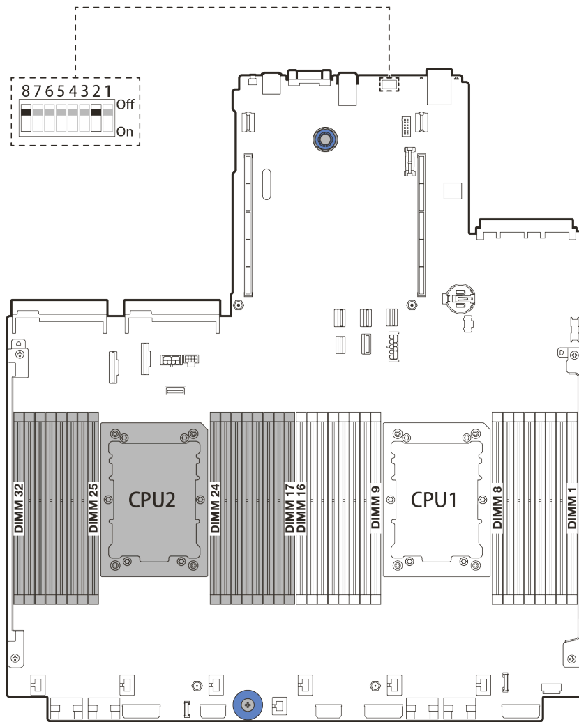
圖例 13. 主機板上的 SW8 開關區塊
