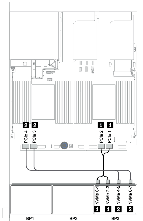
圖例 116. NVMe 纜線佈線 (兩個處理器)
