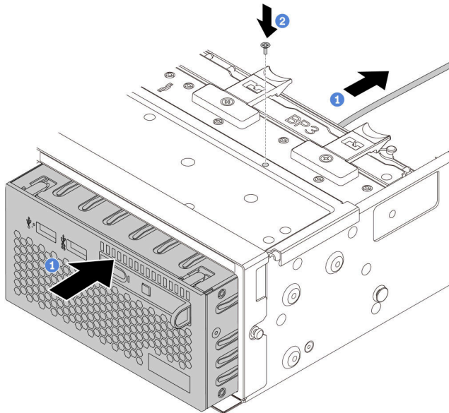
圖例 214. 安裝正面 I/O 模組
