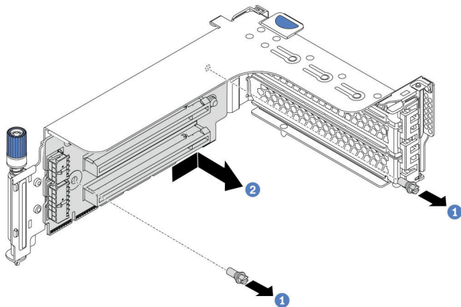
圖例 264. 卸下擴充卡
