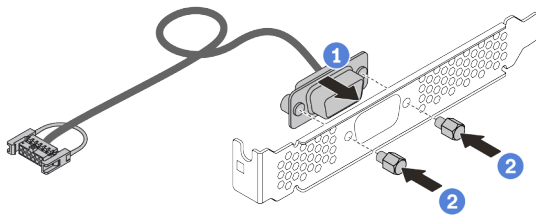
圖例 355. 組裝序列埠模組
