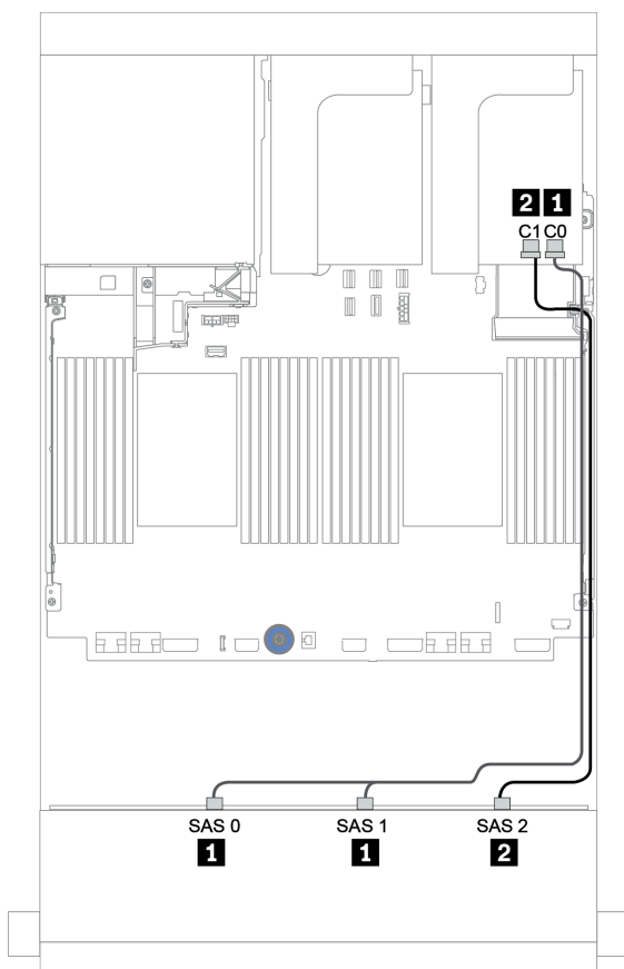
圖例 150. 配置為一個 16i RAID/HBA 配接卡的 12 x 3.5 吋 SAS/SATA 的纜線佈線
