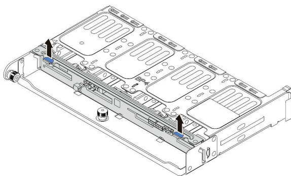
圖例 314. 卸下後方 8 x 2.5 吋硬碟背板
