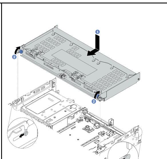
圖例 326. 安裝 4 x 3.5 吋背面框架
