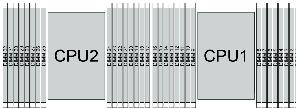
圖例 193. 主機板上的記憶體模組插槽
