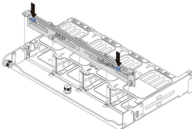
圖例 316. 安裝 8 x 2.5 吋後方硬碟背板
