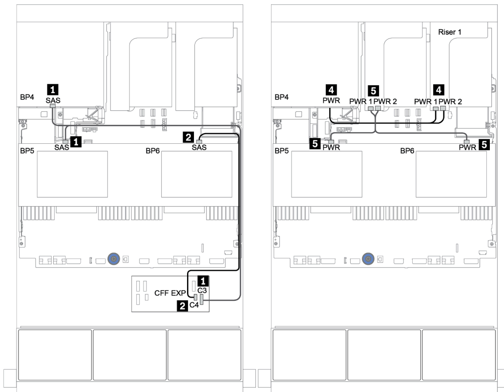
圖例 56. 兩個 4 x 2.5 吋 SAS/SATA 中間背板和一個 4 x 2.5 吋 SAS/SATA 後方背板的纜線佈線
