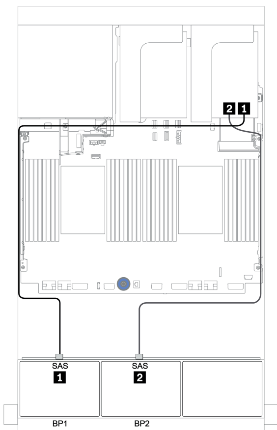
圖例 101. 配置為一個 8i/16i RAID/HBA 配接卡和一個三模式 8i RAID 配接卡的 8 x 2.5 吋 SAS/SATA + 8 x 2.5 吋 AnyBay 的纜線佈線
