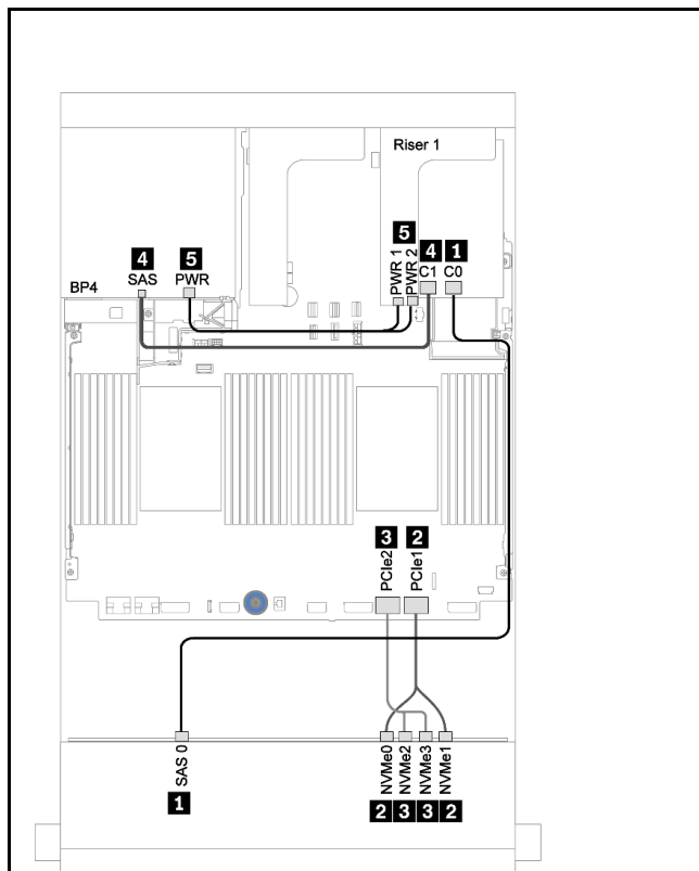
圖例 191. 包含 RAID 930/9350-8i 配接卡的纜線佈線
