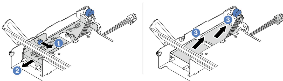
圖例 303. 卸下 RAID 快閃記憶體電源模組
