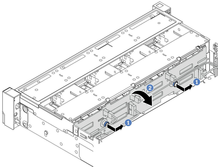
圖例 207. 卸下 3.5 吋硬碟背板
