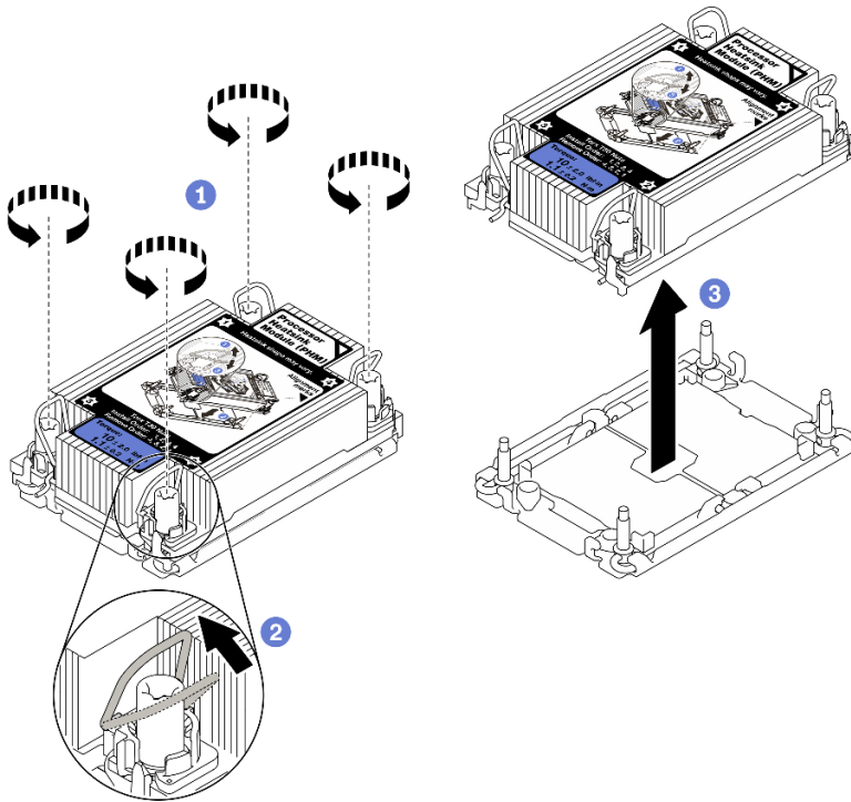
圖例 275. 卸下 PHM
