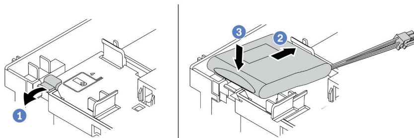
圖例 301. 安裝 RAID 快閃記憶體電源模組 (在空氣擋板上)
