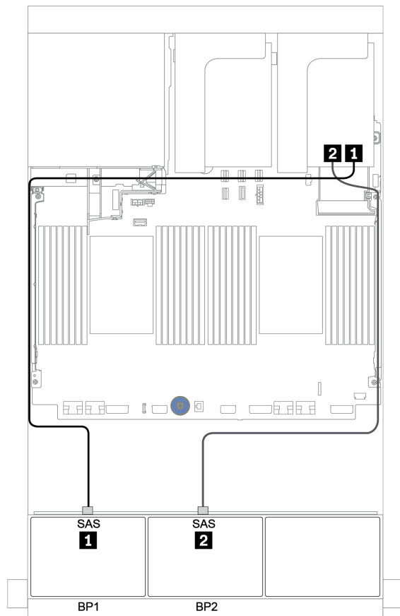
圖例 38. 配置為兩個 8i RAID/HBA 配接卡或一個 16i/32i RAID/HBA 配接卡的 16 x 2.5 吋 SAS/SATA 的纜線佈線
