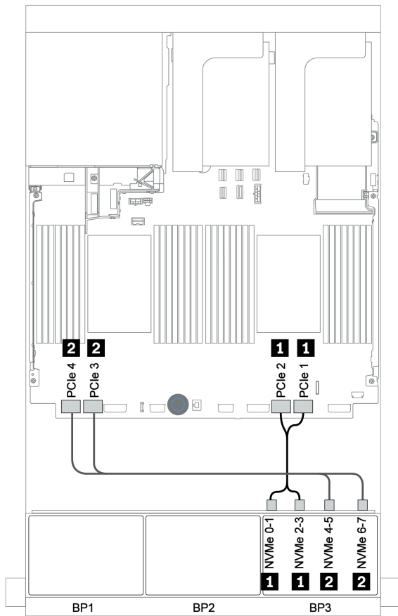
圖例 122. NVMe 纜線佈線
