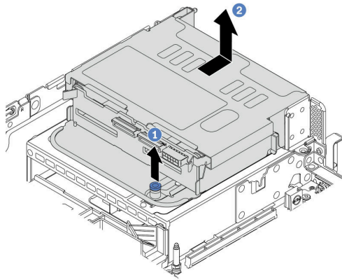
圖例 311. 卸下 4 x 2.5 吋背面框架
