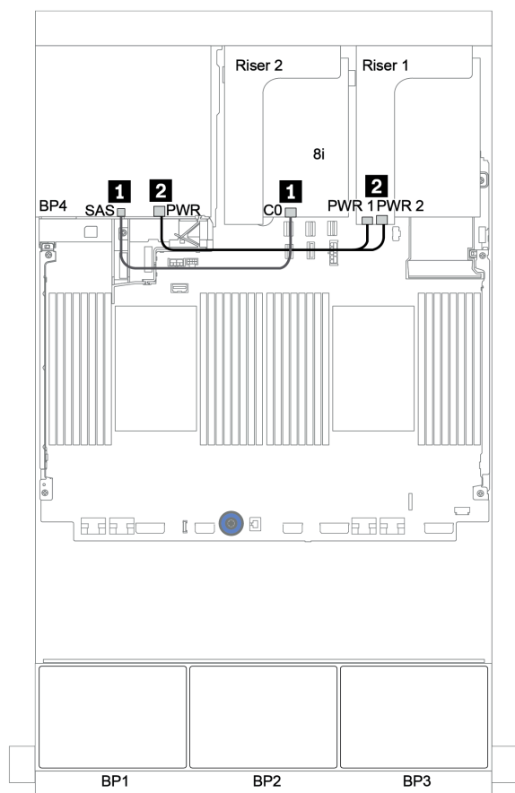
圖例 129. 後方 2.5 吋 SAS/SATA 背板的纜線佈線
