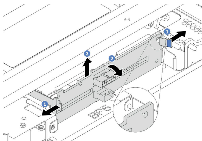
圖例 252. 卸下 2.5 吋中間硬碟背板
