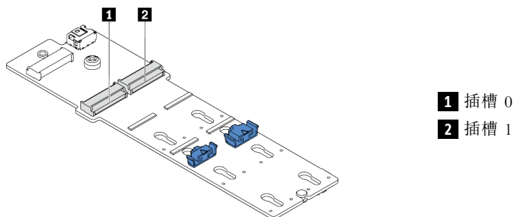
圖例 244. M.2 硬碟插槽
