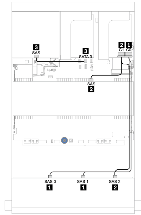
圖例 182. SAS/SATA 纜線佈線
