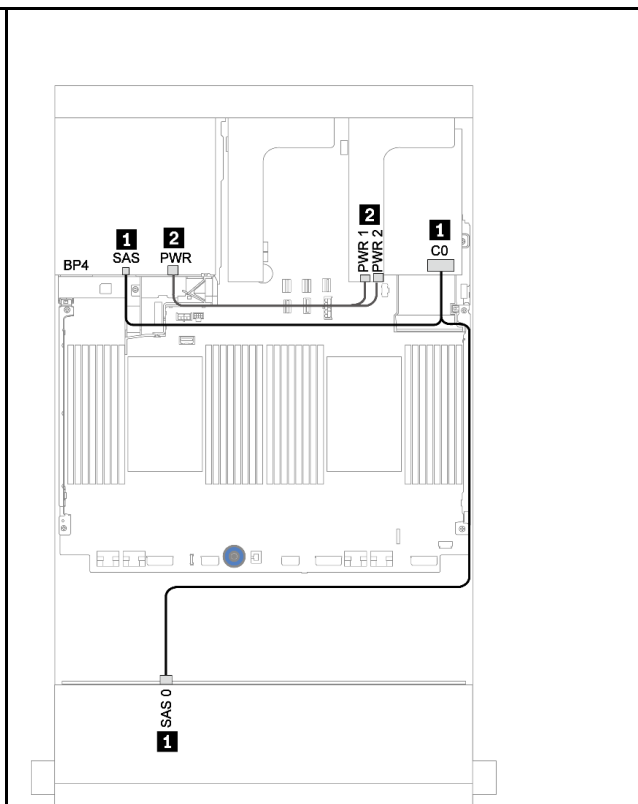
圖例 188. 包含 RAID 940-8i 配接卡的纜線佈線
