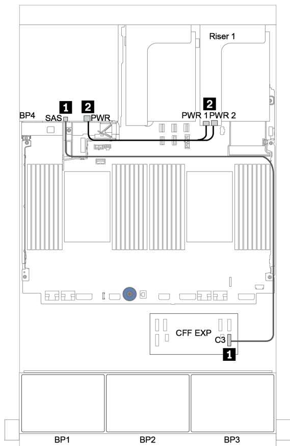
圖例 52. 4 x 2.5 吋 SAS/SATA 後方背板的纜線佈線
