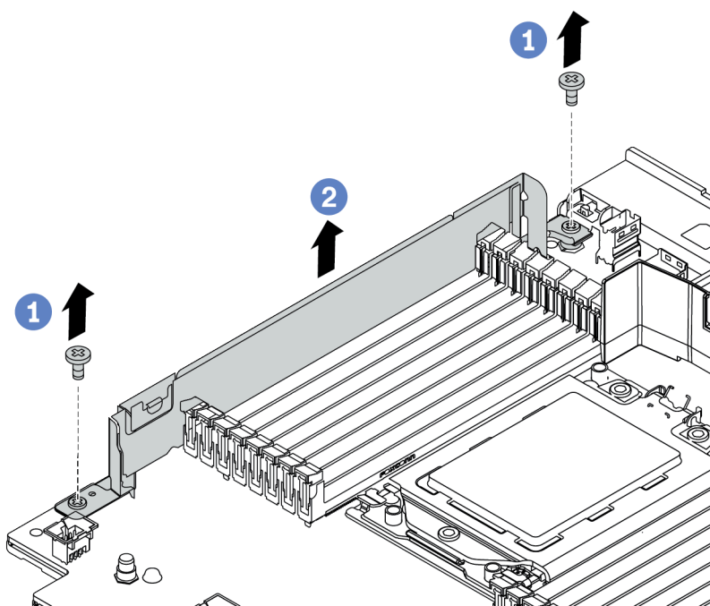
圖例 200. 卸下纜線壁托架
