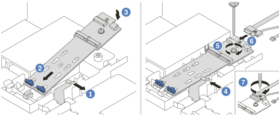
圖例 247. M.2 背板安裝
