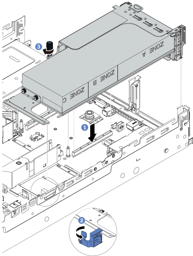
圖例 223. 安裝擴充卡組件
