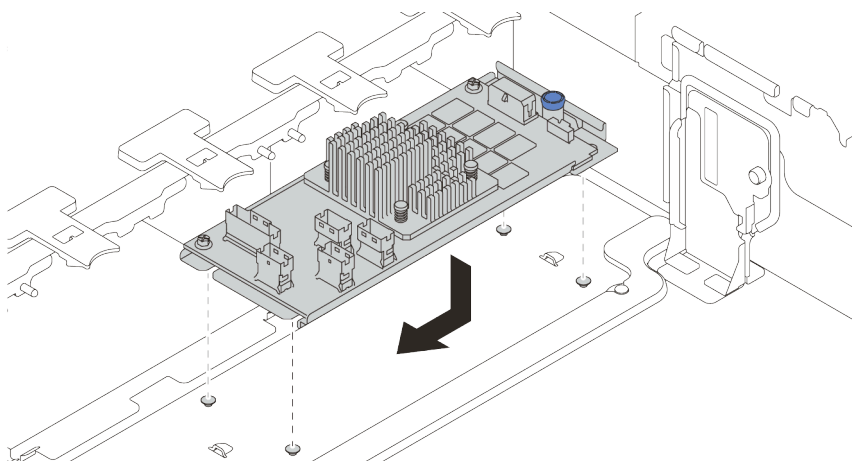
圖例 235. 安裝內部 CFF 配接卡
