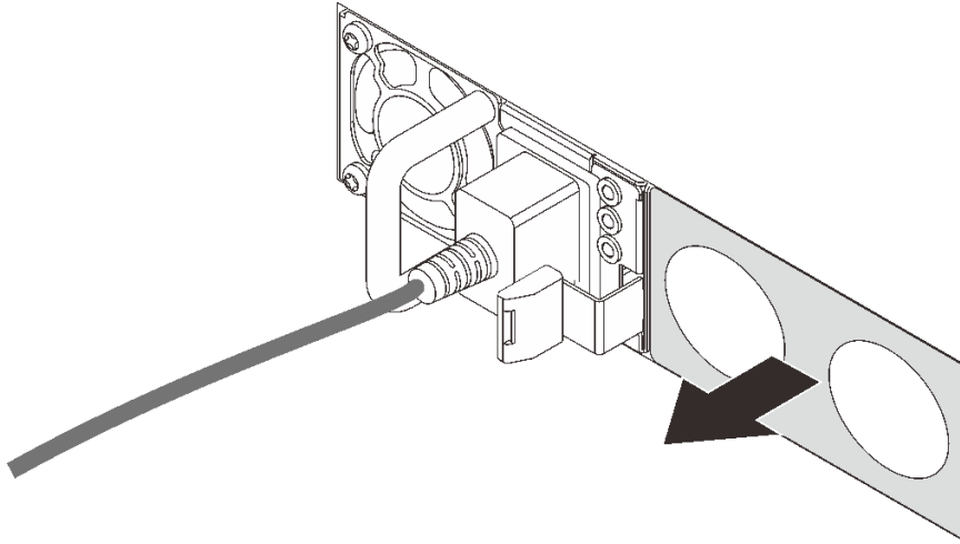
圖例 271. 卸下熱抽換電源供應器填充板
