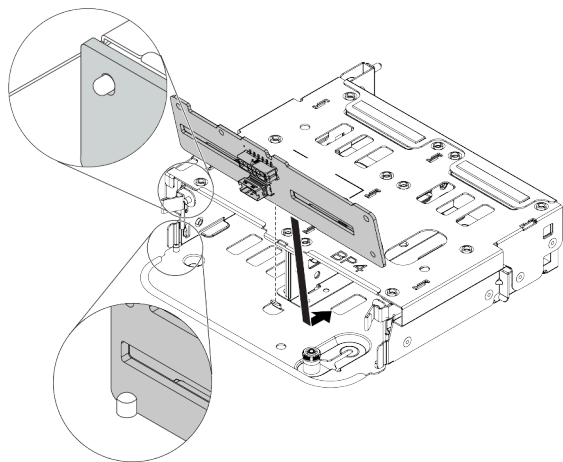
圖例 315. 安裝 4 x 2.5 吋後方硬碟背板
