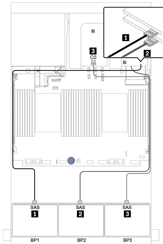
圖例 81. 配置為三個三模式 8i RAID 配接卡的 24 x 2.5 吋 AnyBay 的纜線佈線
