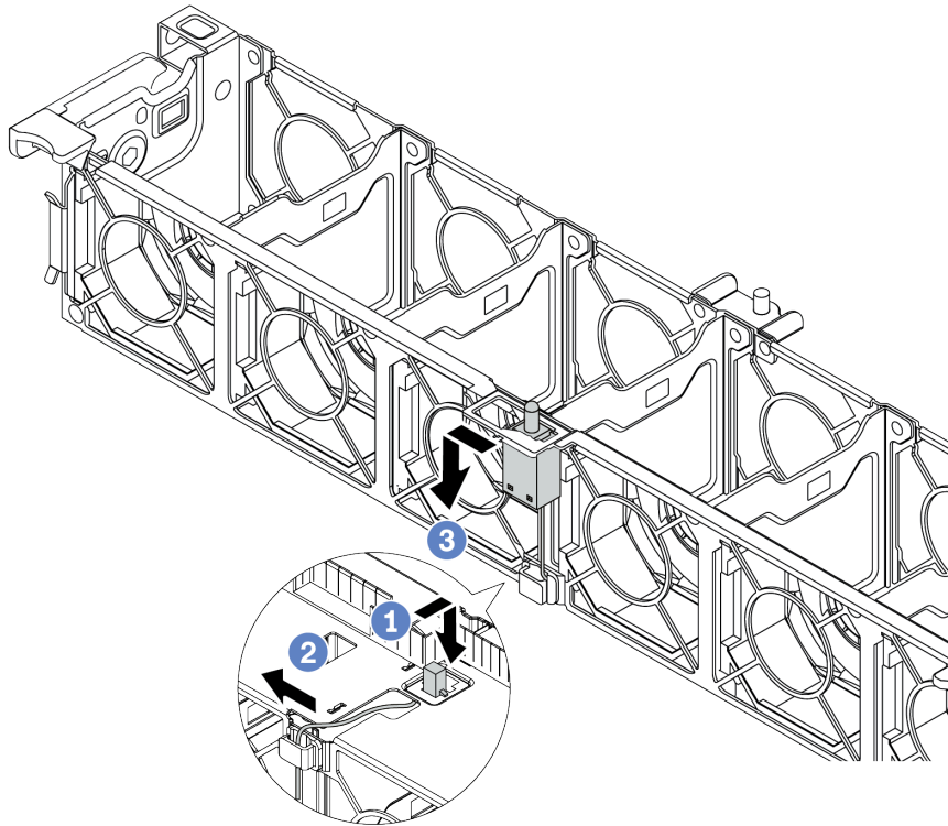
圖例 236. 卸下入侵開關
