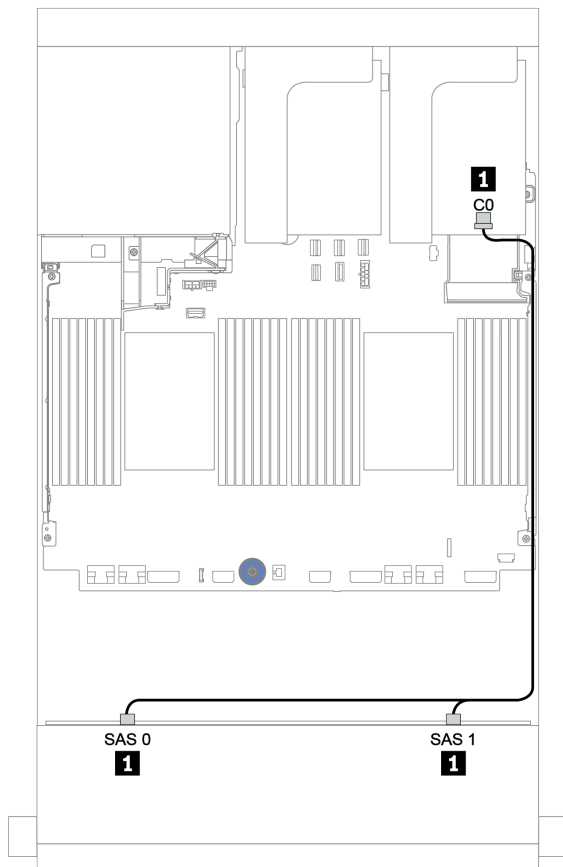
圖例 148. 配置為一個 8i RAID/HBA 配接卡的 8 x 3.5 吋 SAS/SATA 的纜線佈線
