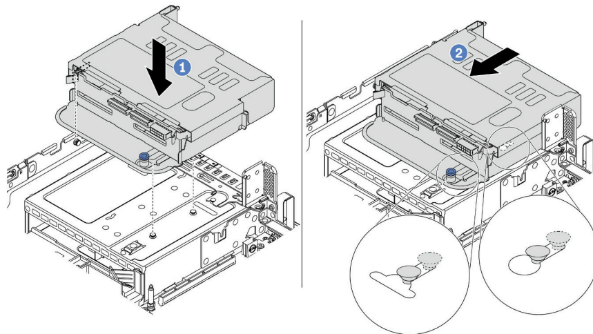
圖例 317. 安裝 4 x 2.5 吋背面框架
