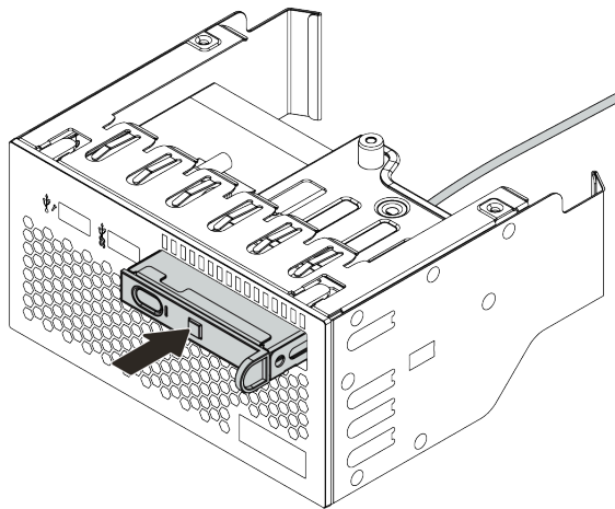
圖例 215. 安裝整合式診斷面板
