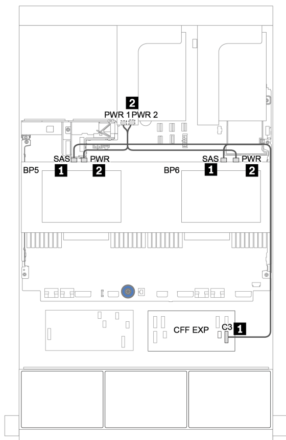
圖例 54. 兩個中間 4 x 2.5 SAS/SATA 背板的纜線佈線
