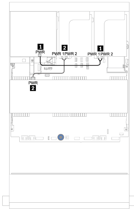
圖例 168. 電源線佈線
