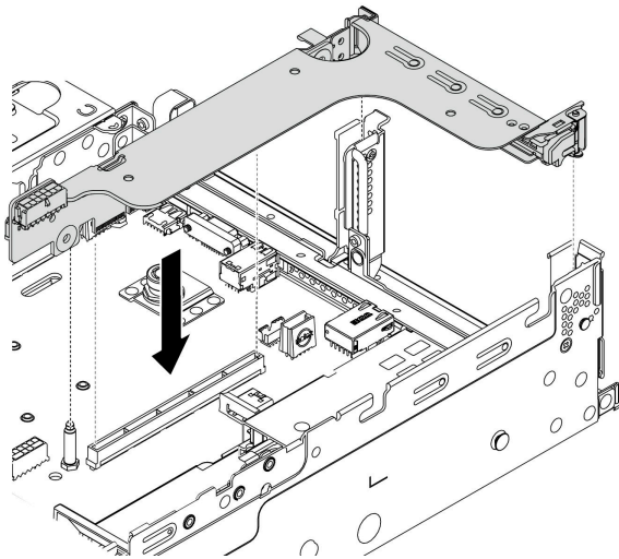
圖例 357. 安裝擴充卡組件
