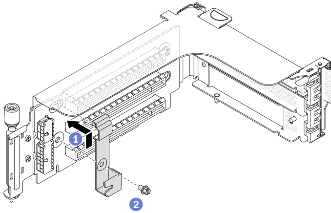
圖例 335. 安裝 7 公釐框架固定夾
