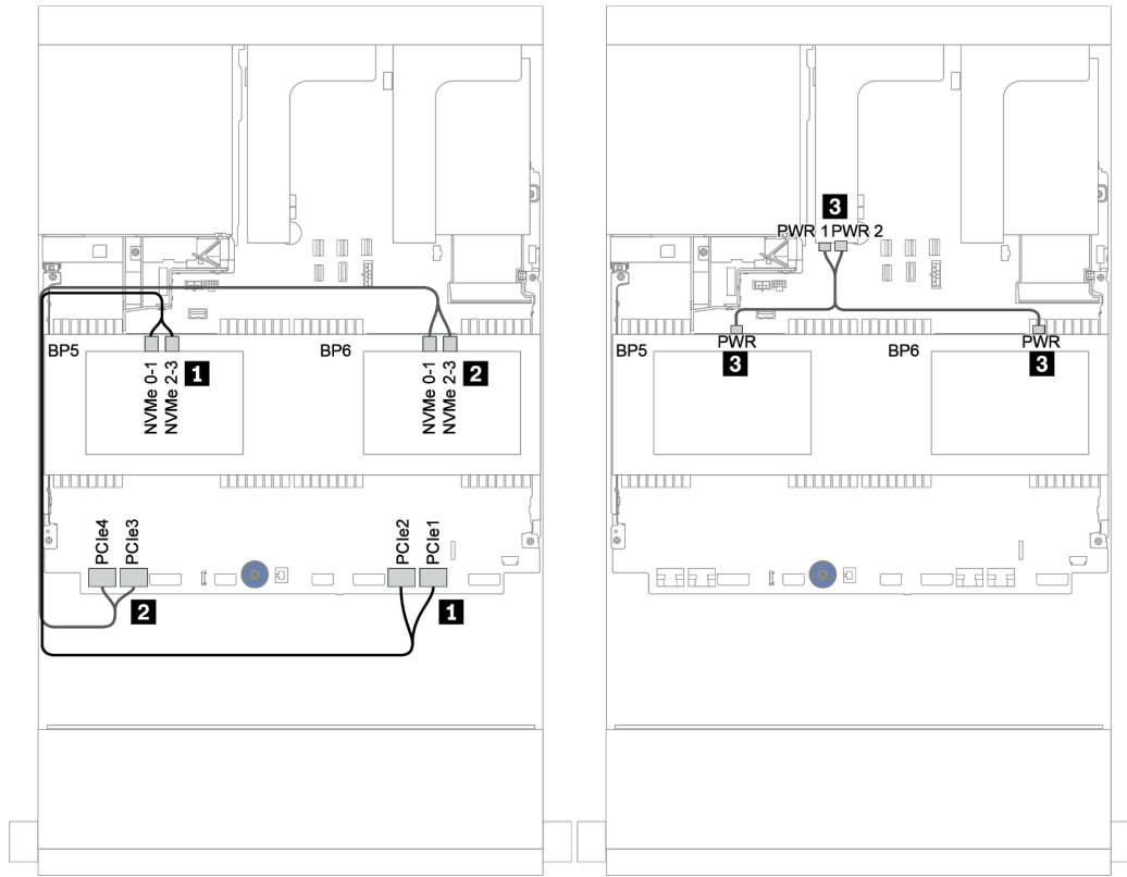
圖例 163. 兩個 4 x 2.5 吋 NVMe 中間硬碟背板的纜線佈線
