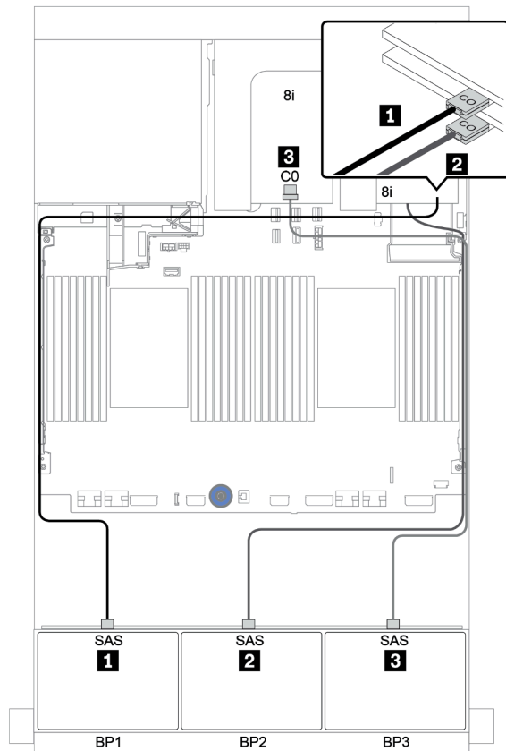
圖例 127. SAS/SATA 纜線佈線
