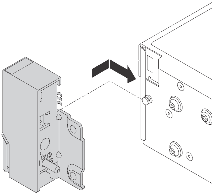
圖例 289. 機架門鎖安裝
