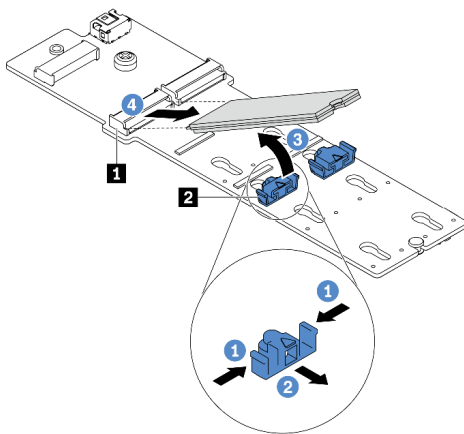
圖例 243. 卸下 M.2 硬碟
