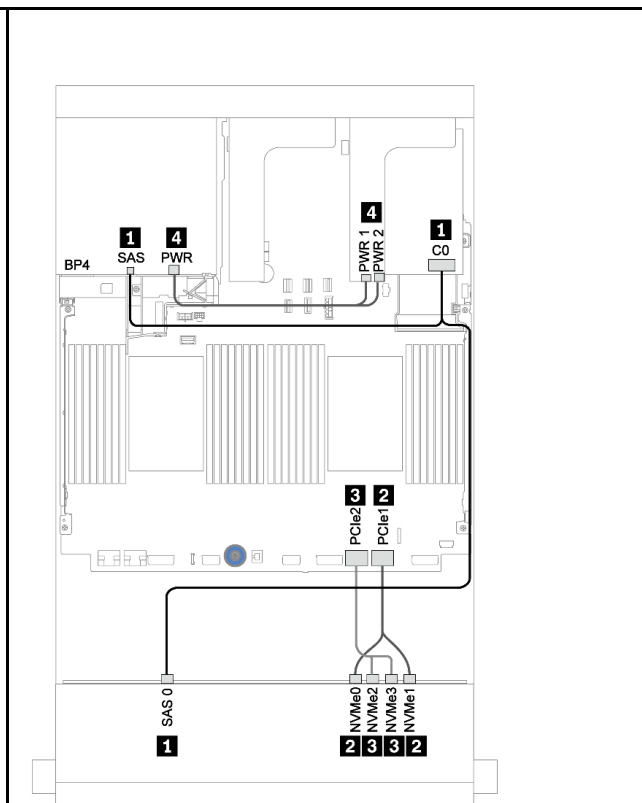
圖例 192. 包含 RAID 940-8i 配接卡的纜線佈線
