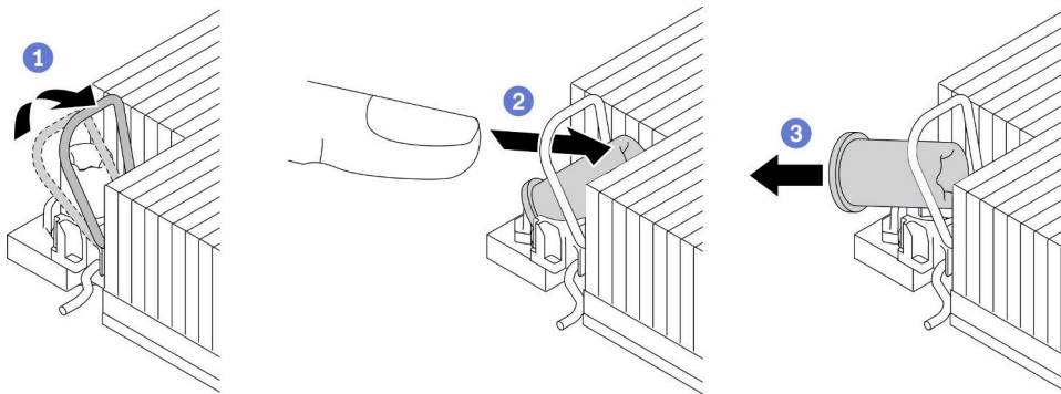
圖例 225. 從散熱槽卸下 Torx T30 螺帽
