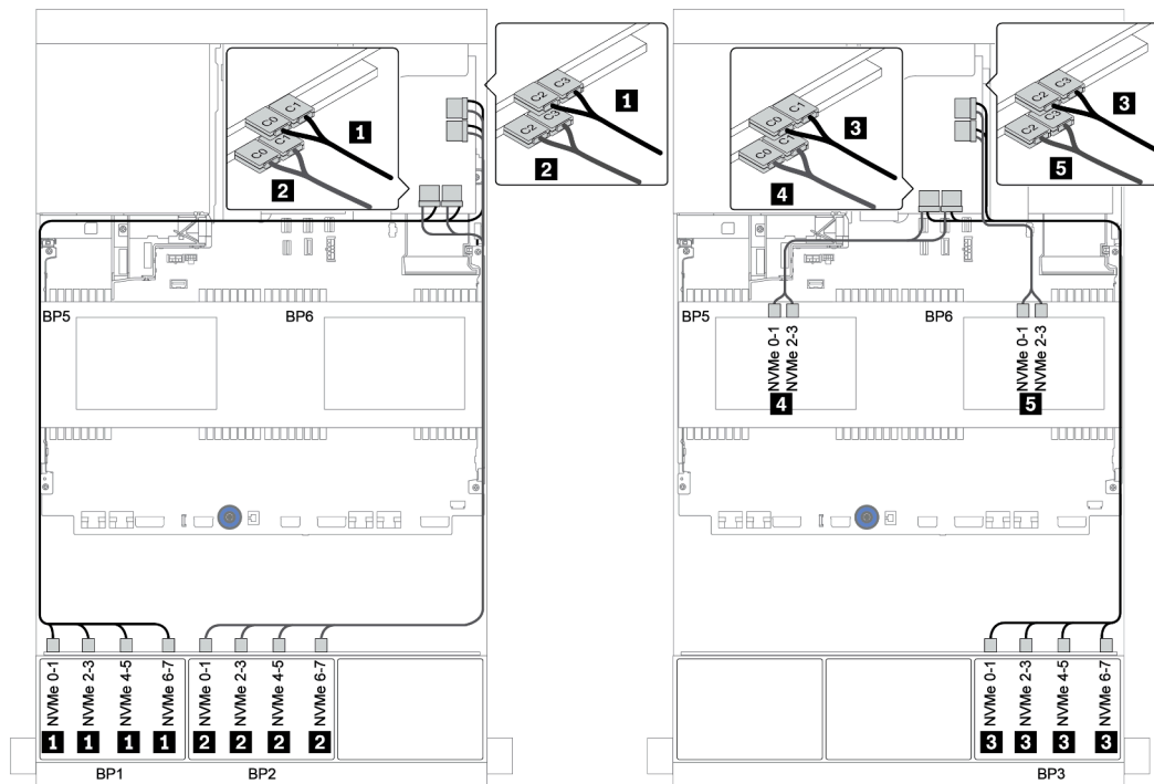
圖例 67. 配置為四個交換器卡的 32 x 2.5 吋 NVMe 的纜線佈線
