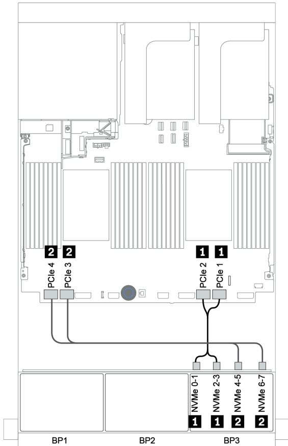
圖例 120. NVMe 纜線佈線 (兩個處理器)
