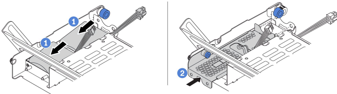
圖例 304. 安裝 RAID 快閃記憶體電源模組
