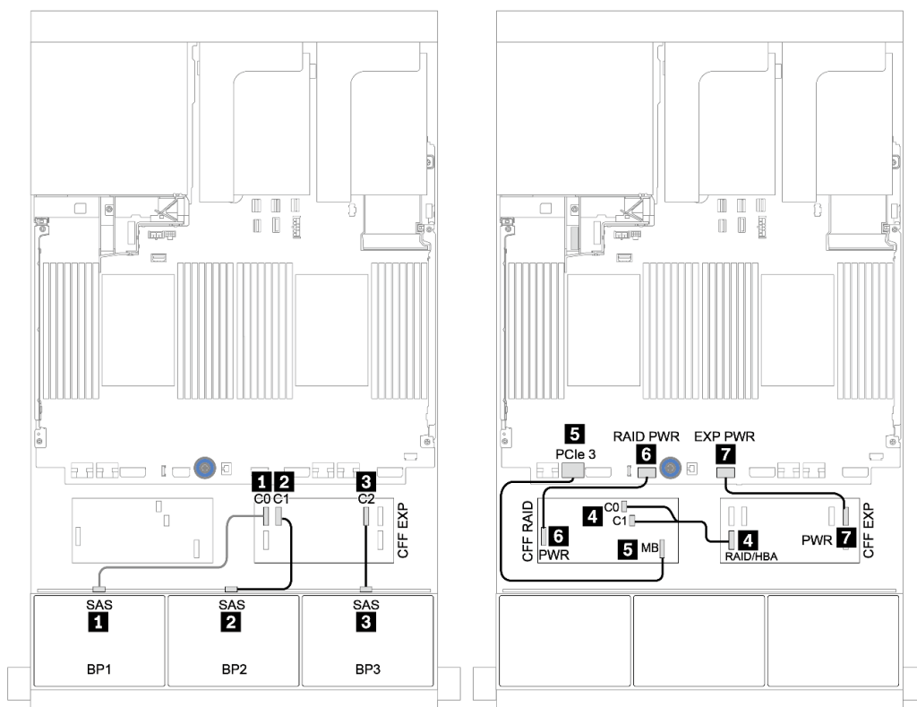
圖例 59. 配置為一個 CFF 16i RAID/HBA 配接卡和一個 CFF 擴充器的 24 x 2.5 吋 SAS/SATA 的纜線佈線
