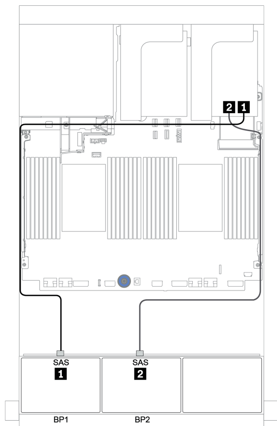
圖例 79. 配置為兩個三模式 8i RAID 配接卡的 16 x 2.5 吋 AnyBay 的纜線佈線
