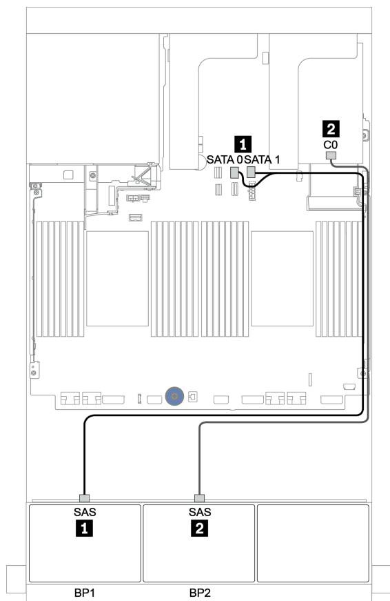
圖例 100. 配置為一個三模式 8i RAID 配接卡的 8 x 2.5 吋 SAS/SATA + 8 x 2.5 吋 AnyBay 的纜線佈線
