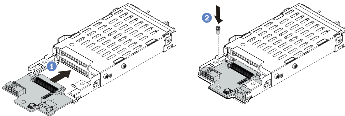
圖例 333. 7 公釐硬碟背板安裝 (底部)
