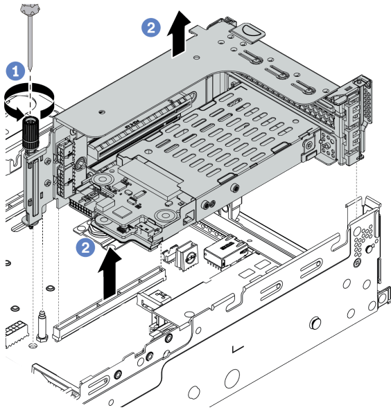
圖例 328. 卸下擴充卡組件
