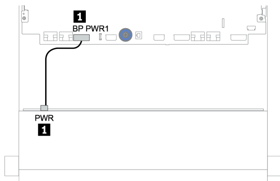
圖例 145. 8 x 3.5 吋 SAS/SATA 硬碟背板的電源線佈線
