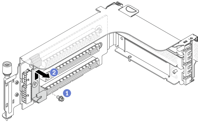
圖例 330. 卸下 7 公釐框架固定夾
