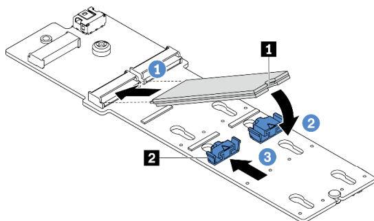
圖例 245. M.2 硬碟安裝
