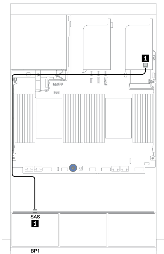
圖例 34. 配置為一個 8i/16i RAID/HBA 配接卡的 8 x 2.5 吋 SAS/SATA 的纜線佈線
