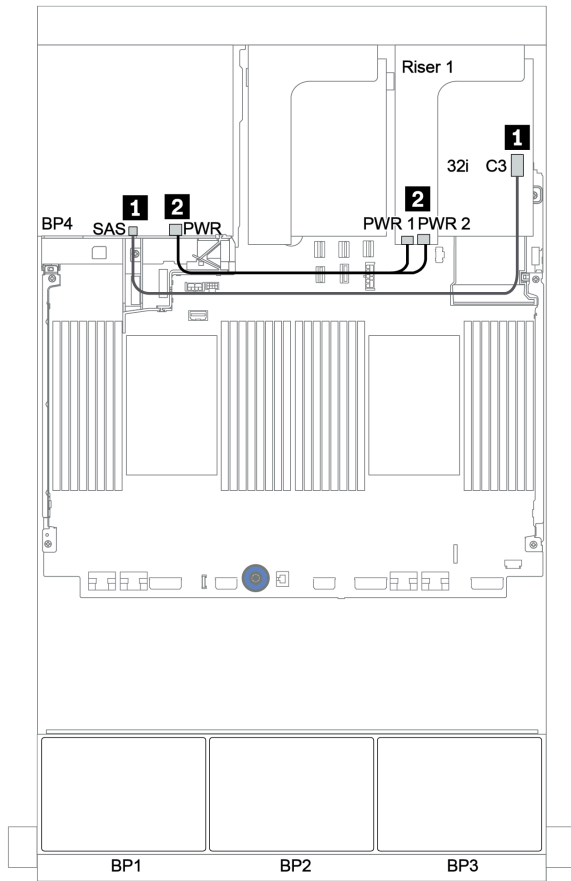
圖例 132. 後方 4 x 2.5 吋 SAS/SATA 背板的纜線佈線
