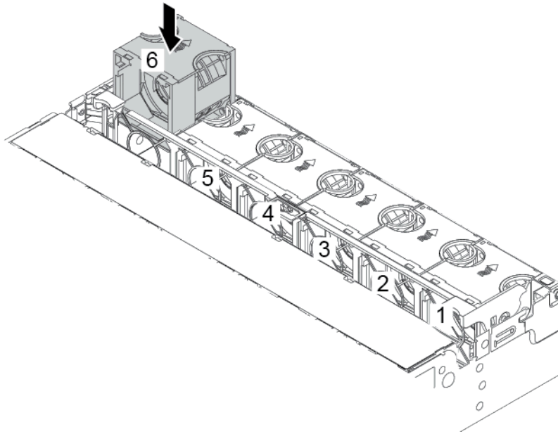
圖例 348. 安裝系統風扇
