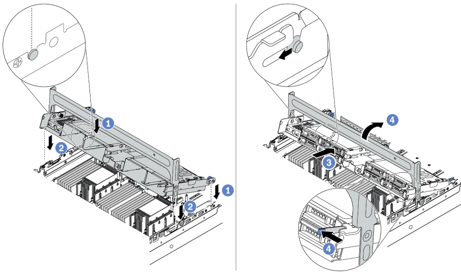
圖例 256. 安裝中間框架和硬碟
