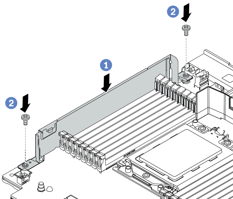
圖例 201. 安裝纜線壁托架
