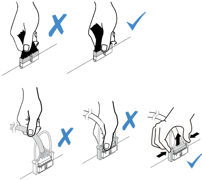
圖例 233. 從主機板拔掉纜線
