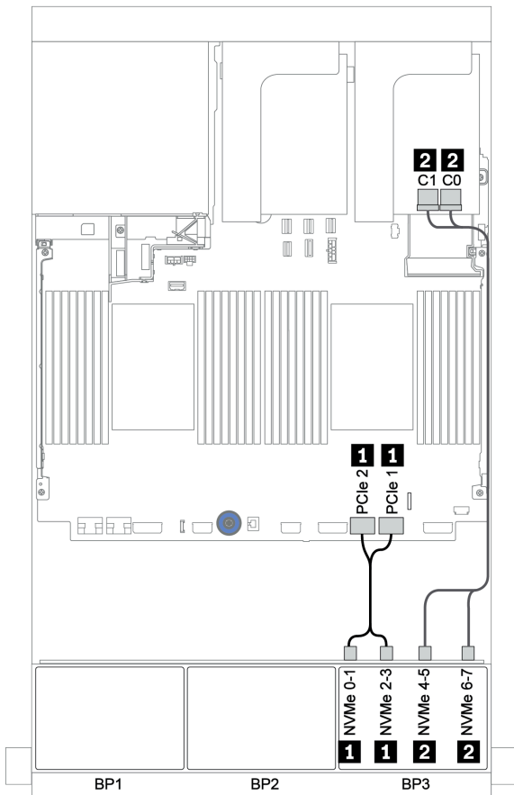
圖例 143. NVMe 纜線佈線 (一個處理器)
