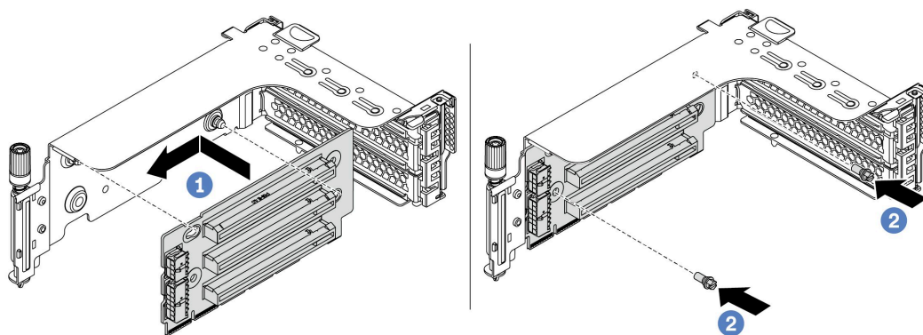
圖例 265. 擴充卡安裝
