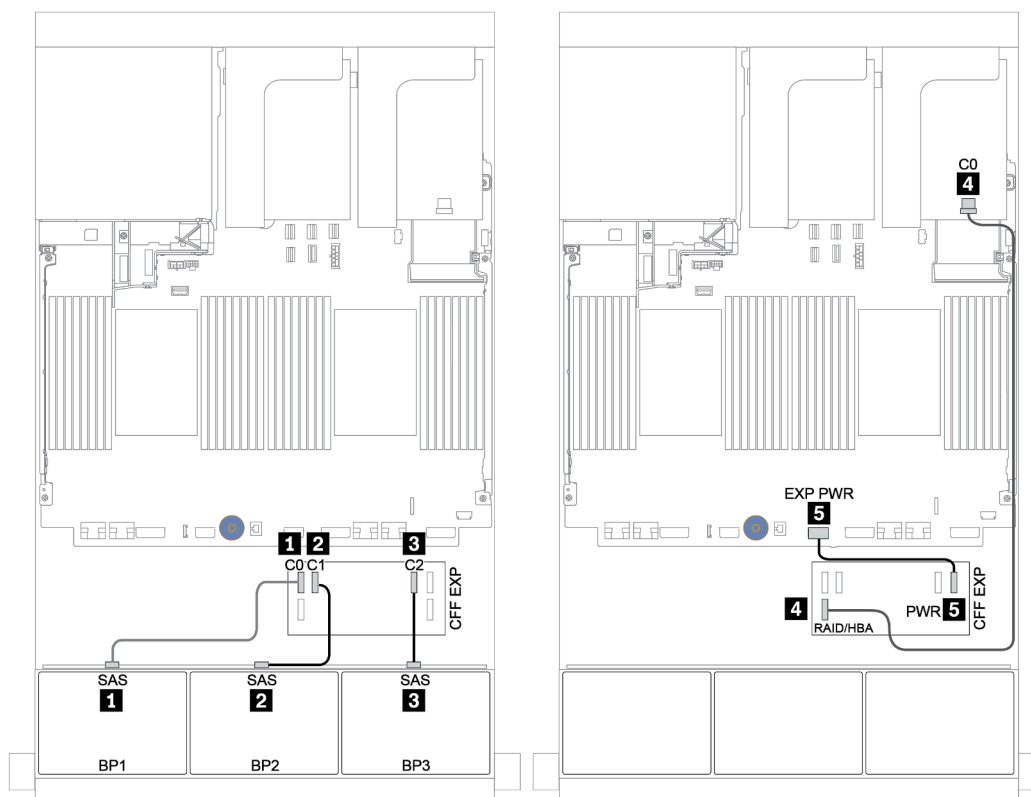
圖例 142. SAS/SATA 纜線佈線
