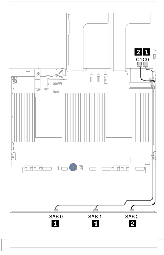
圖例 162. 配備一個 16i RAID/HBA 配接卡的 12 x 3.5 吋 SAS/SATA 前方背板的纜線佈線
