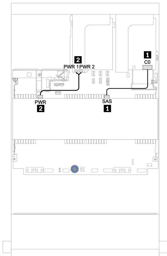
圖例 161. 4 x 3.5 吋 SAS/SATA 中間背板的纜線佈線
