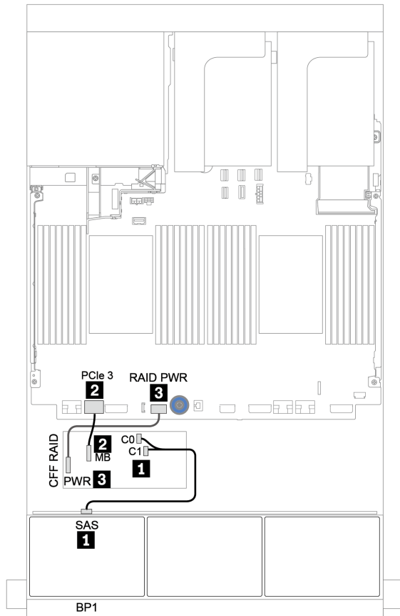
圖例 35. 配置為一個 CFF 8i RAID 配接卡的 8 x 2.5 吋 SAS/SATA 的纜線佈線
