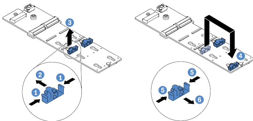
圖例 246. 調整 M.2 固定器
