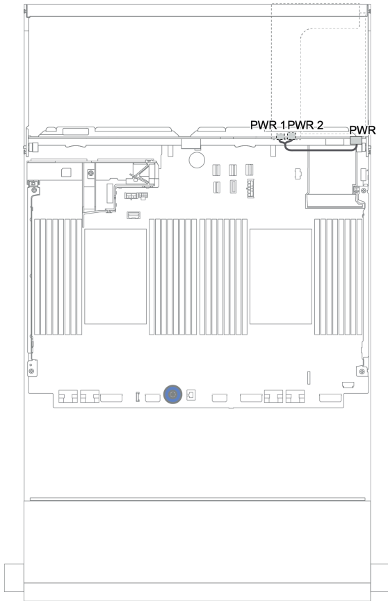
圖例 178. 後方背板的電源線佈線
