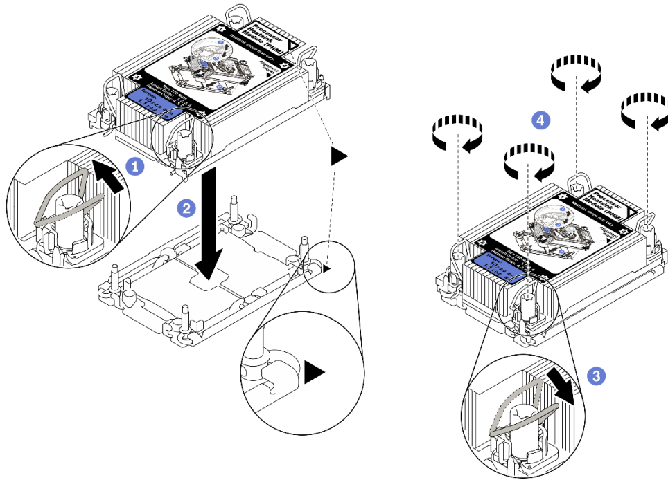
圖例 283. 安裝 PHM
