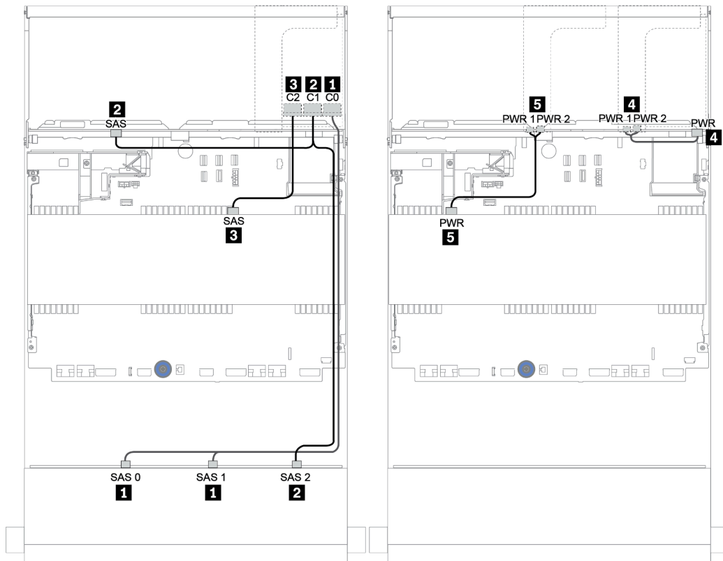
圖例 166. 配置為一個 32i RAID 配接卡的 12 x 3.5 吋 SAS/SATA + 4 x 3.5 吋 SAS/SATA + 4 x 3.5 吋 SAS/SATA 的纜線佈線
