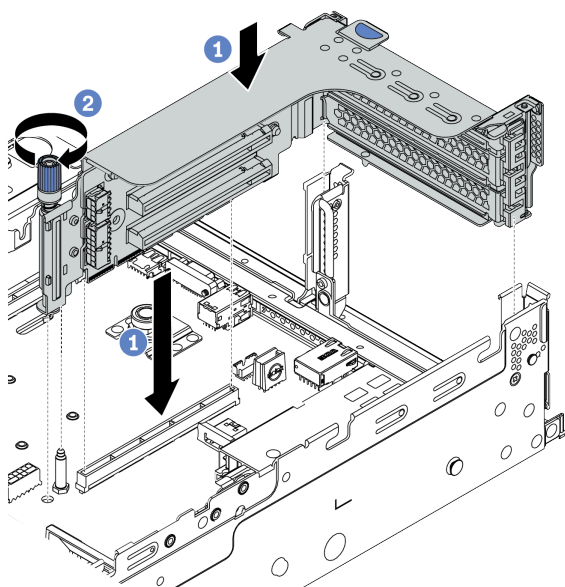
圖例 267. 安裝擴充卡組件
