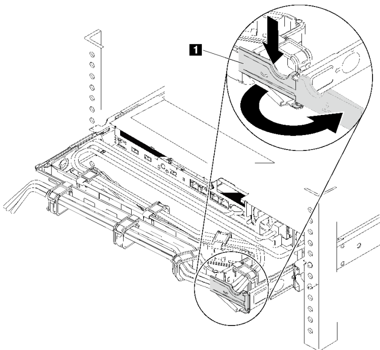
圖例 268. 調整 CMA
