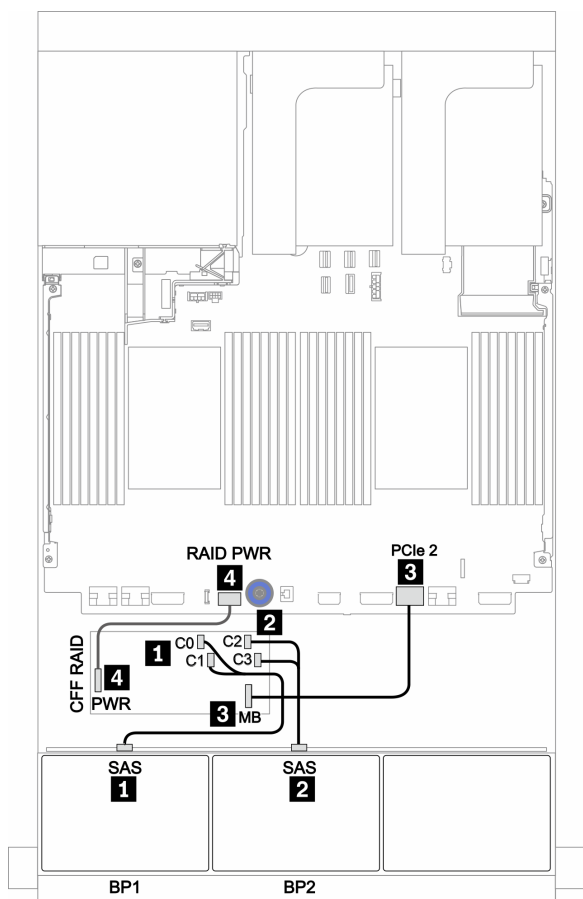
圖例 80. 配置為一個三模式 CFF 16i RAID 配接卡的 16 x 2.5 吋 AnyBay 的纜線佈線
