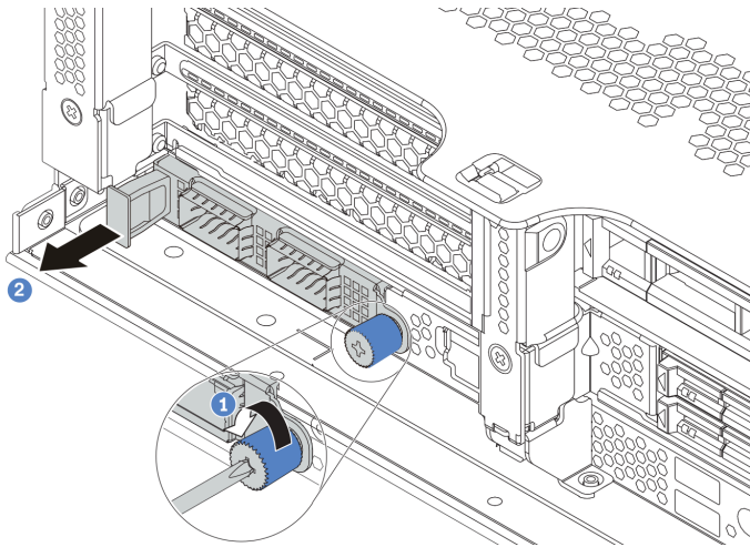
圖例 257. 卸下 OCP 3.0 乙太網路配接卡
