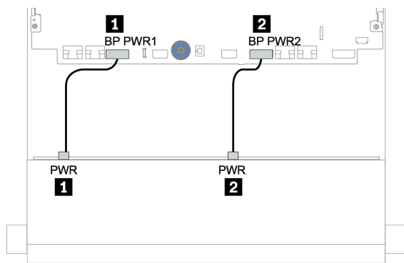
圖例 146. 12 x 3.5 吋硬碟背板的電源線佈線
