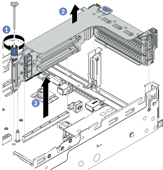
圖例 262. 卸下擴充卡組件
