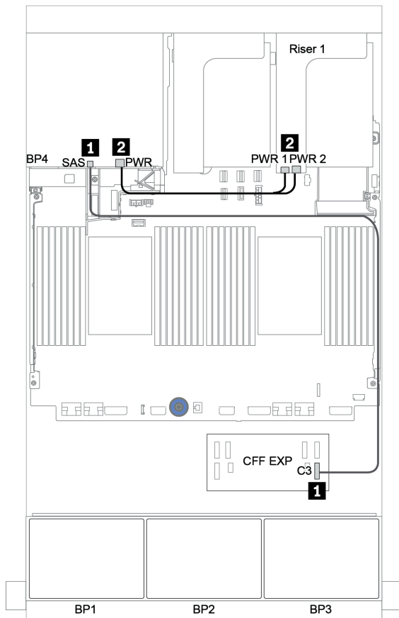
圖例 135. 後方 4 x 2.5 吋 SAS/SATA 背板的纜線佈線
