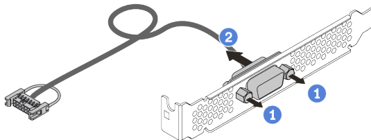
圖例 354. 拆卸序列埠模組
