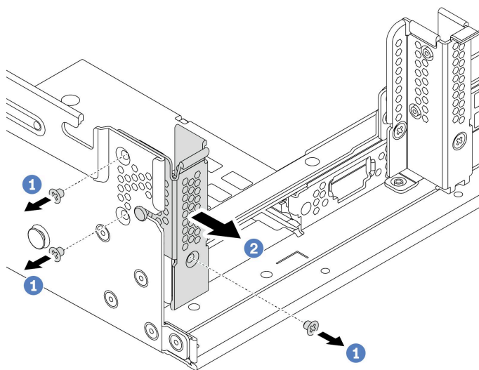
圖例 305. 卸下 A1 後壁托架 (左)
