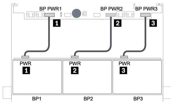
圖例 32. 8 x 2.5 吋硬碟背板的電源線連接
