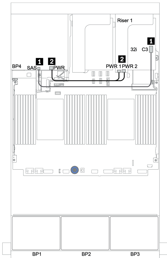
圖例 48. 後方 4 x 2.5 吋 SAS/SATA 背板的纜線佈線
