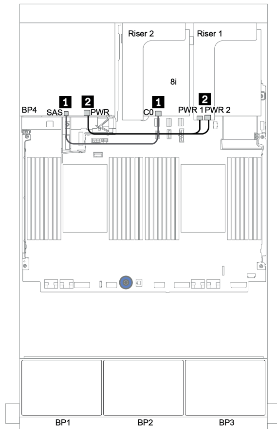
圖例 46. 後方 4 x 2.5 吋 SAS/SATA 背板的纜線佈線
