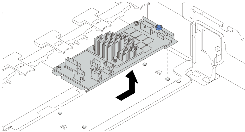
圖例 234. 卸下內部 CFF 配接卡
