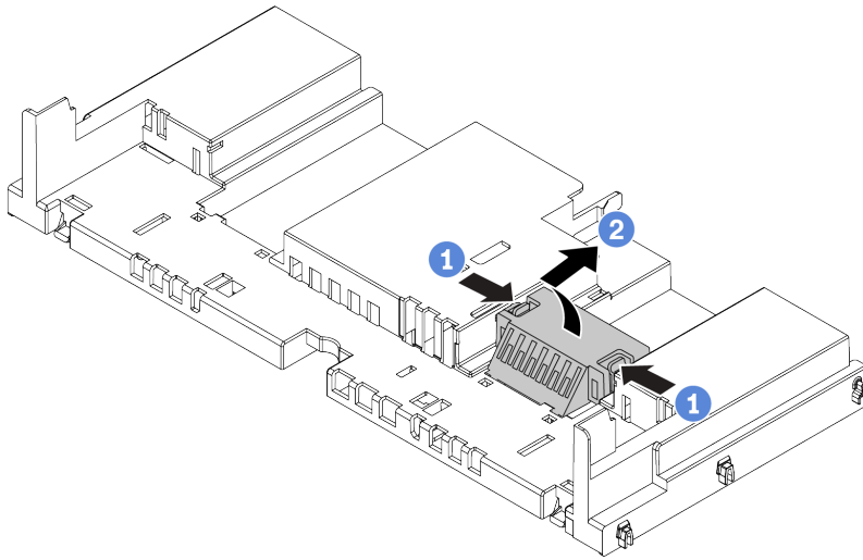
圖例 197. 卸下空氣擋板填充板
