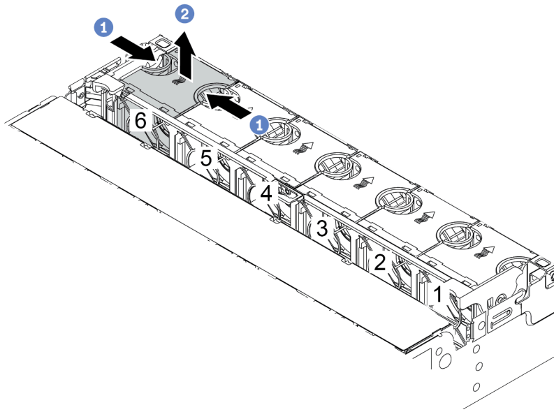
圖例 347. 卸下系統風扇
