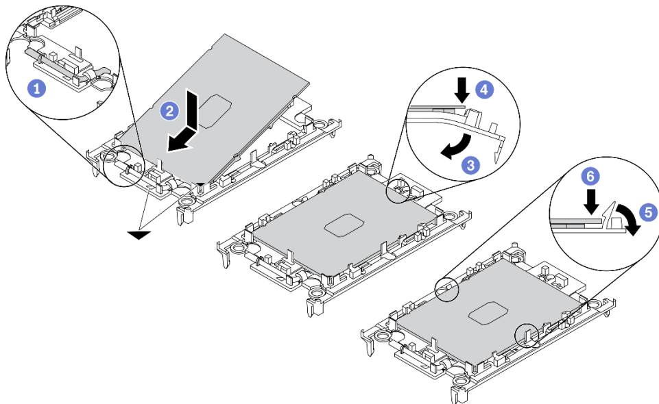
圖例 280. 安裝處理器支架
