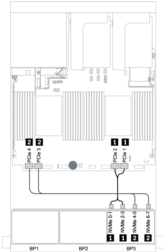
圖例 128. NVMe 纜線佈線 (兩個處理器)
