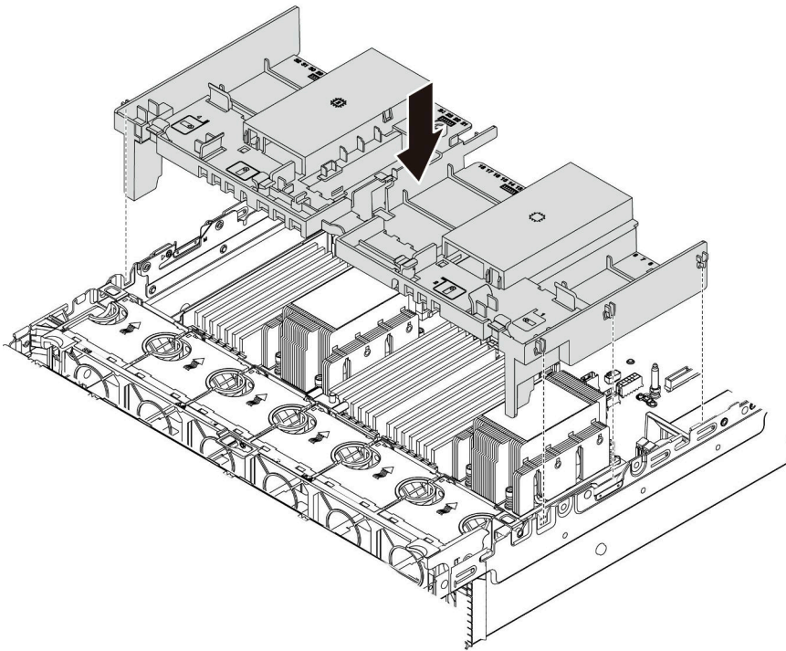
圖例 199. 安裝標準空氣擋板
