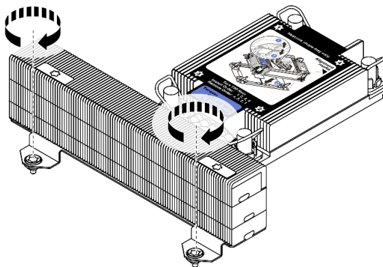
圖例 284. 鎖緊 T 形散熱槽螺絲
