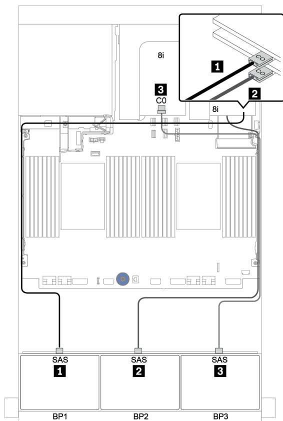
圖例 107. 配置為一個 8i/16i RAID/HBA 配接卡和兩個三模式 8i RAID 配接卡的 8 x 2.5 吋 SAS/SATA + 16 x 2.5 吋 AnyBay 的纜線佈線
