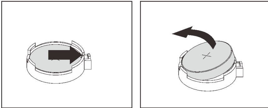
圖例 202. 卸下 CMOS 電池
