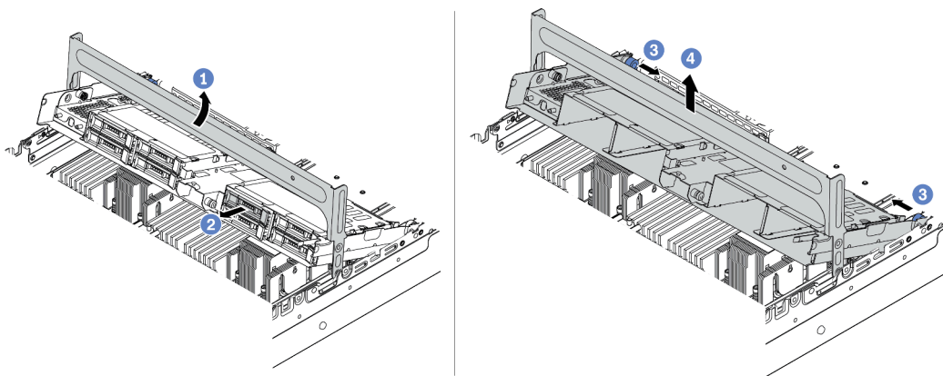
圖例 250. 卸下中間框架和硬碟
