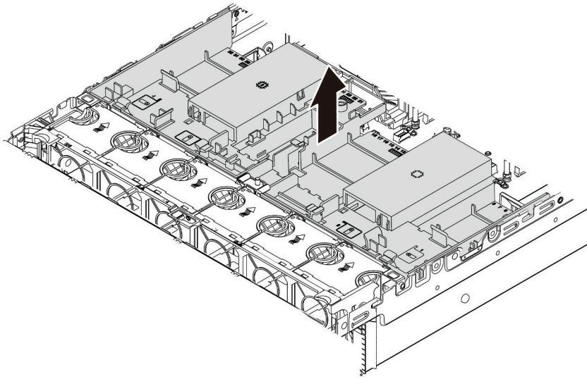
圖例 196. 卸下空氣擋板
