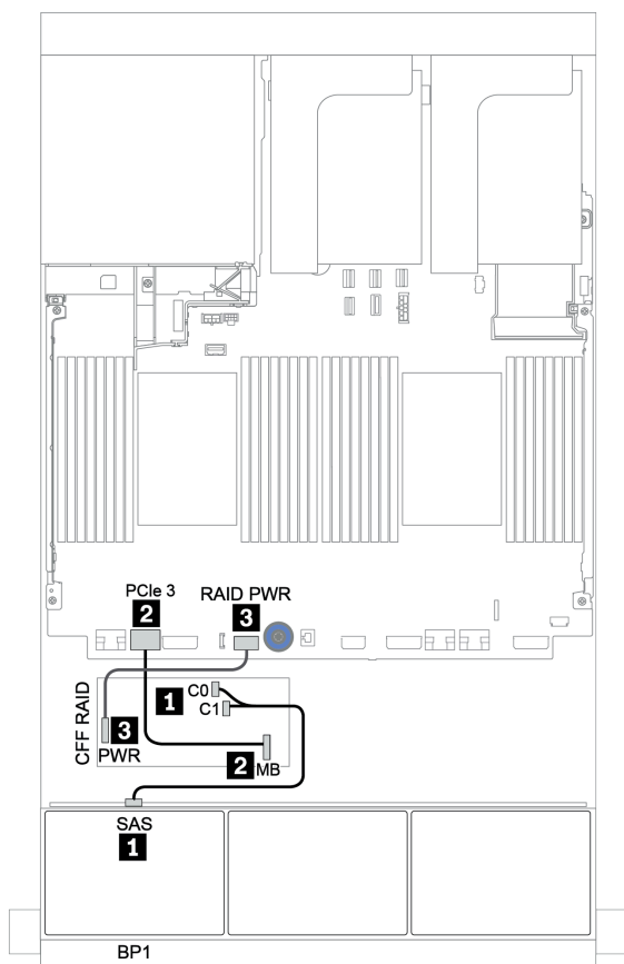
圖例 36. 配置為一個 CFF 16i RAID/HBA 配接卡的 8 x 2.5 吋 SAS/SATA 的纜線佈線
