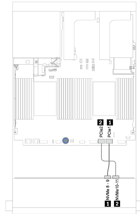
圖例 183. NVMe 纜線佈線
