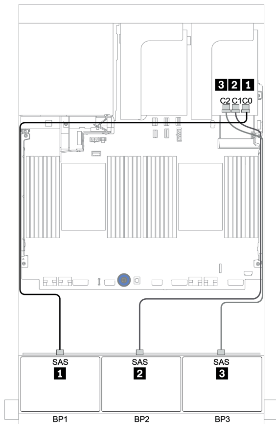
圖例 41. 配置為一個 32i RAID 配接卡的 24 x 2.5 吋 SAS/SATA 的纜線佈線
