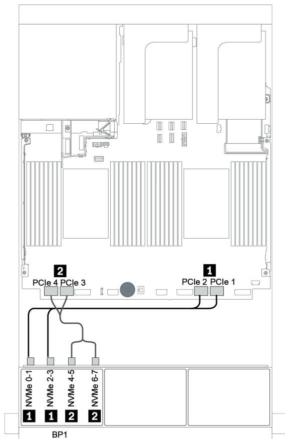
圖例 63. 配置為機載接頭的 8 x 2.5 吋 NVMe 的纜線佈線
