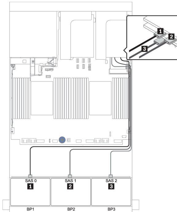
圖例 42. 配置為一個 16i HBA 配接卡和一個 8i RAID 配接卡的 24 x 2.5 吋 SAS/SATA 的纜線佈線
