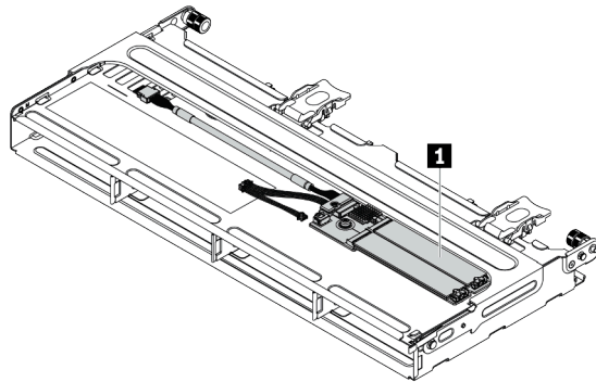
圖例 29. 在 4 x 3.5 中間框架上
