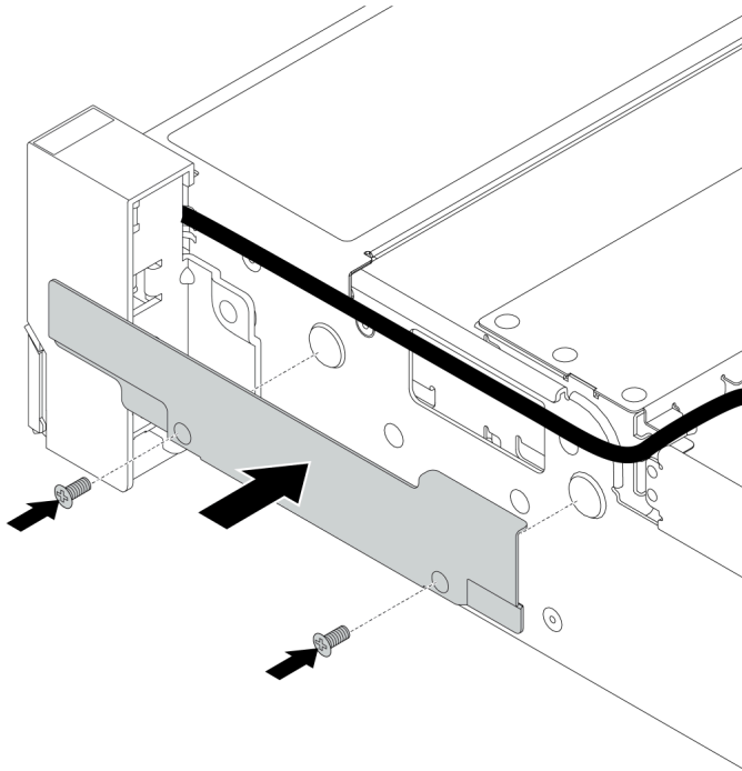
圖例 291. 纜線固定夾安裝
