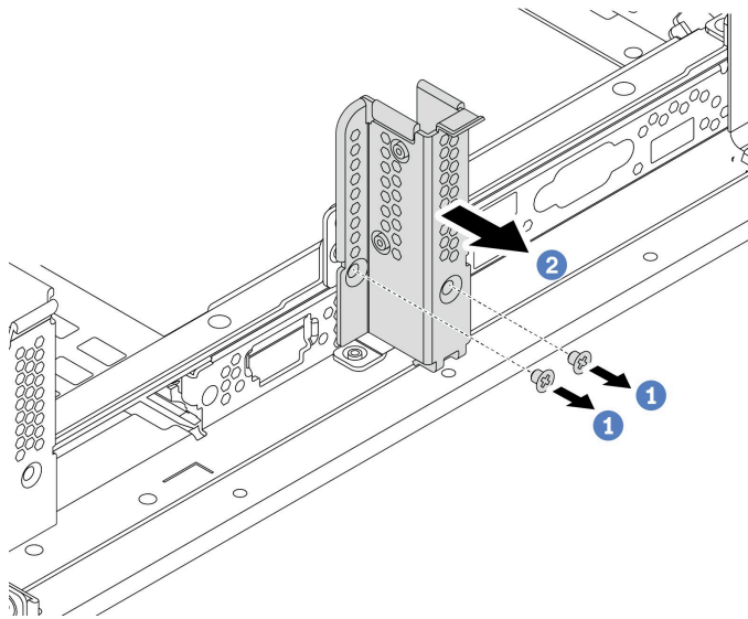
圖例 306. 卸下 B1 後壁托架 (中間)
