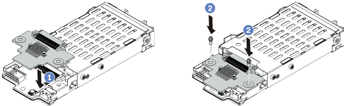
圖例 334. 7 公釐硬碟背板安裝 (頂端)
