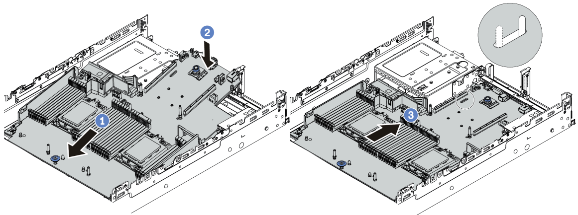
圖例 346. 安裝主機板
