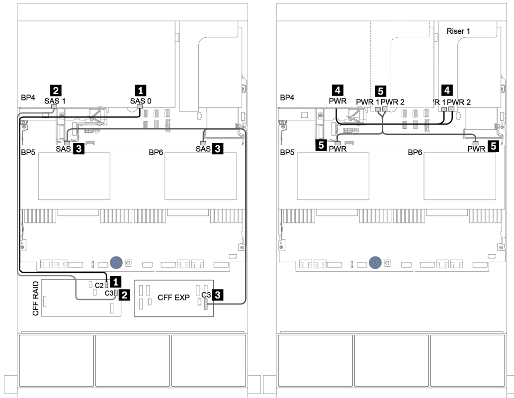
圖例 60. 中間 4 x 2.5 吋 SAS/SATA 背板和後方 8 x 2.5 吋 SAS/SATA 背板的纜線佈線
