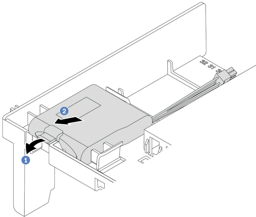
圖例 300. 卸下 RAID 快閃記憶體電源模組
