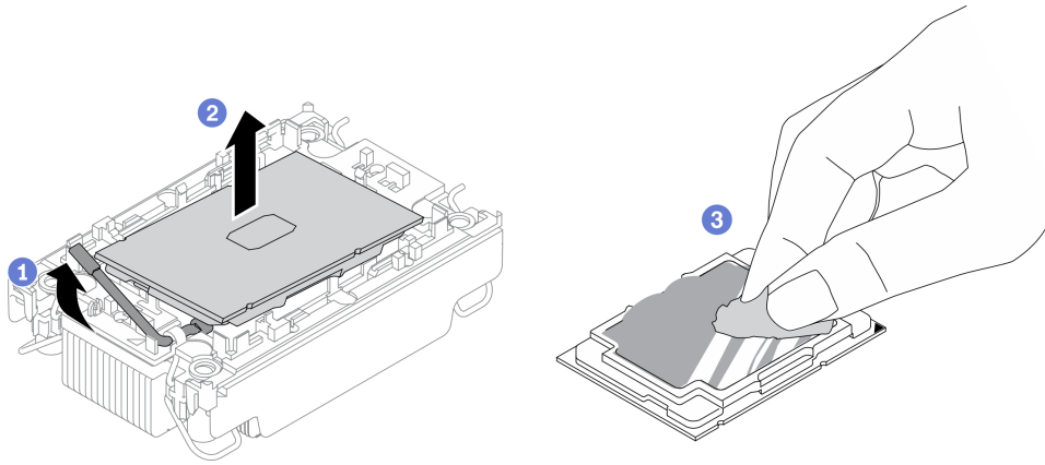
圖例 277. 將處理器與散熱槽和支架分開
