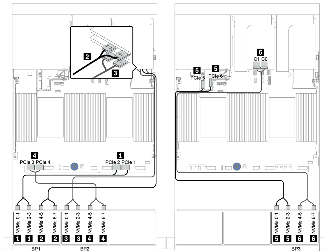
圖例 66. 配置三個重定時器卡的 24 x 2.5 吋 NVMe 的纜線佈線
