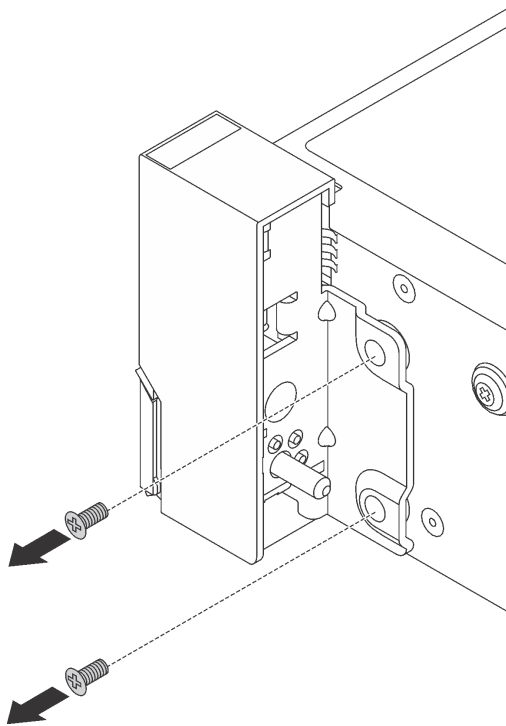
圖例 287. 卸下螺絲
