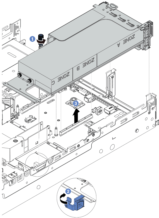
圖例 219. 卸下擴充卡組件
