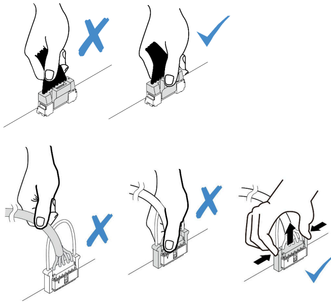
圖例 241. 從主機板拔掉纜線
