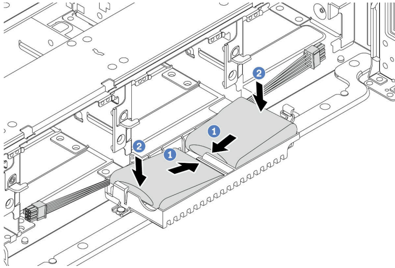
圖例 299. 安裝 RAID 快閃記憶體電源模組
