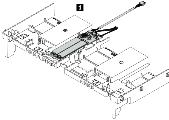
圖例 26. 在標準空氣擋板上
