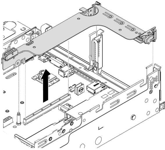
圖例 352. 卸下擴充卡托架
