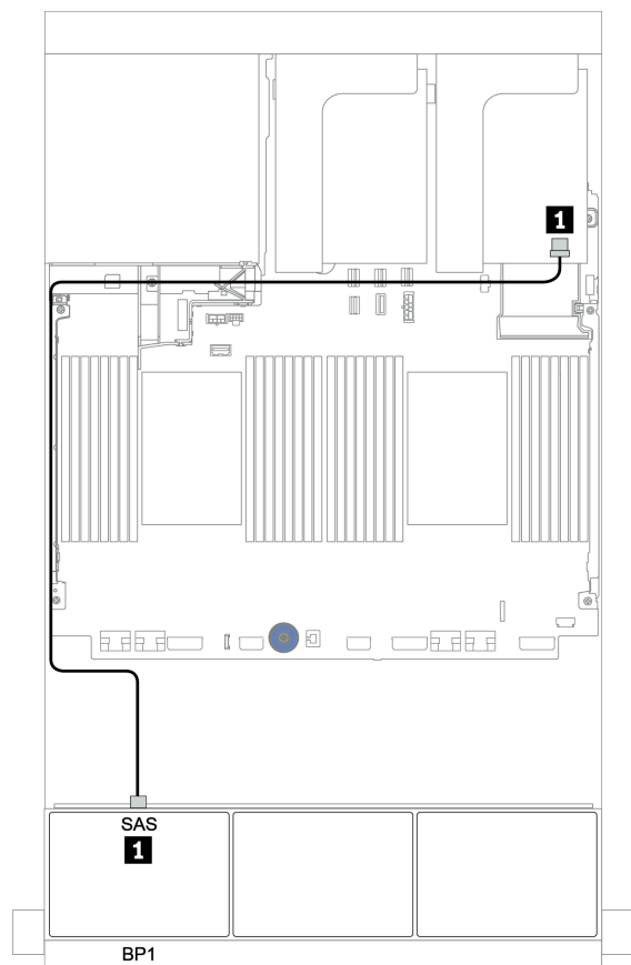
圖例 78. 配置為一個三模式 8i RAID 配接卡的 8 x 2.5 吋 AnyBay 的纜線佈線
