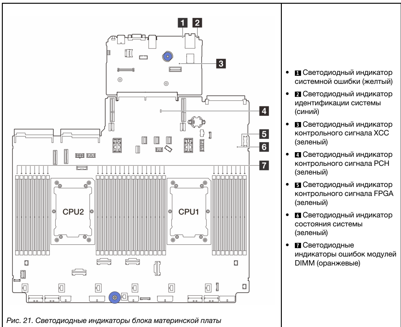
Табл. 30. Светодиодные индикаторы блока материнской платы
