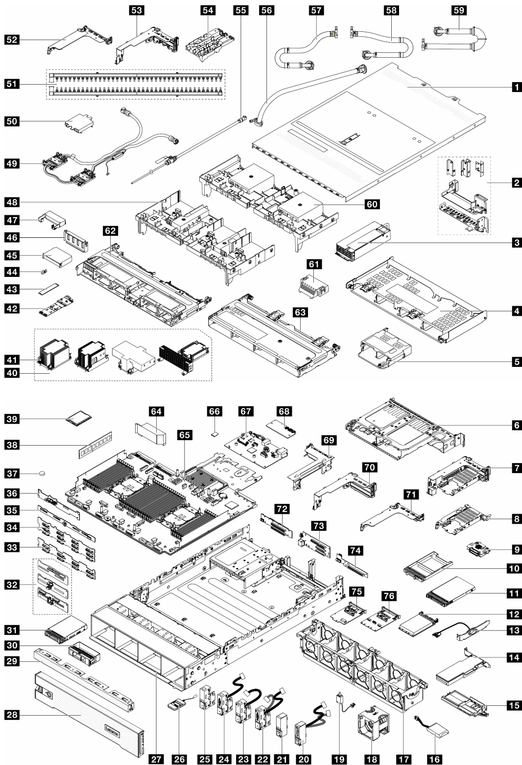
Рис. 25. Компоненты сервера (рама с отсеками для 3,5-дюймовых дисков)
