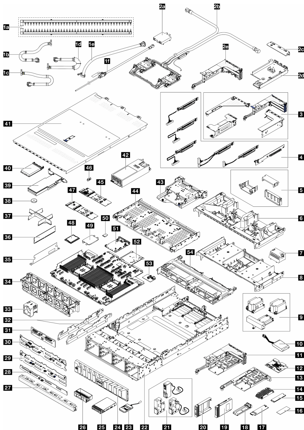
Figure 20. Composants serveur (châssis avec baie d'unité de 3,5 pouces)
