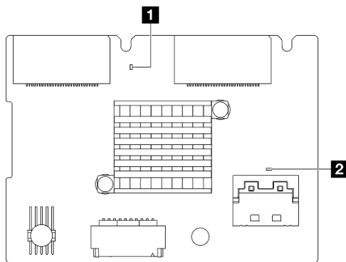
Figure 16. Voyants du fond de panier M.2 arrière
