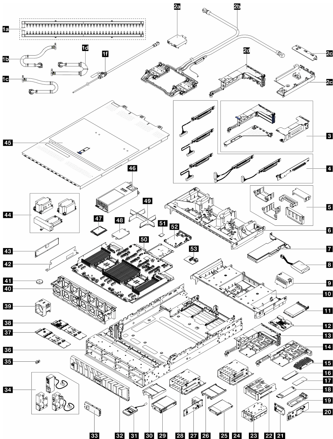
Figure 21. Composants serveur (châssis de baie E3.S)
