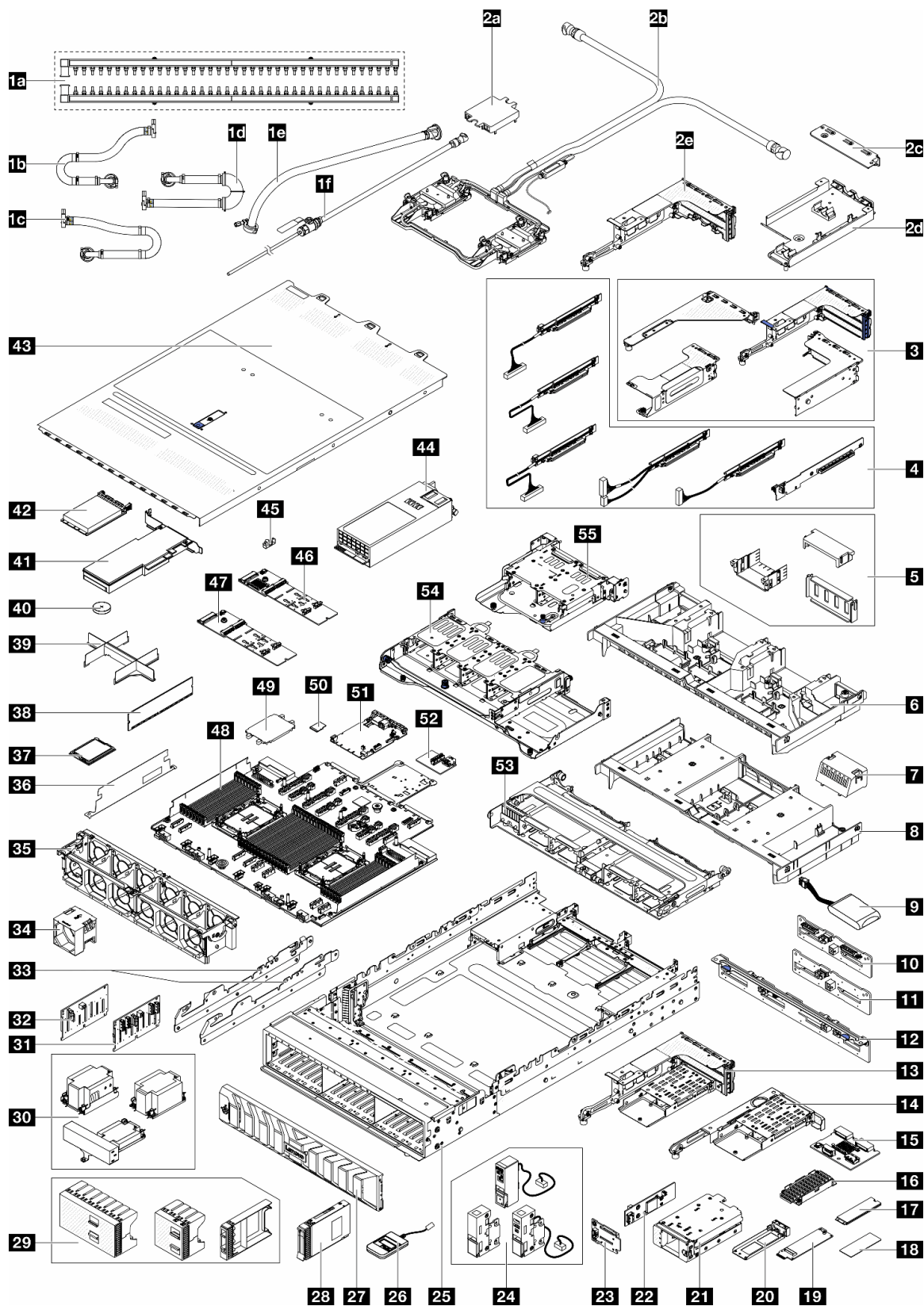
Figure 19. Composants serveur (châssis avec baie d'unité de 2,5 pouces)
