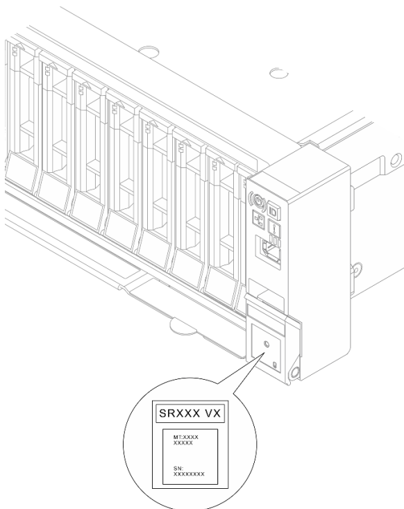
Figure 22. Emplacement de l'étiquette d'identification
