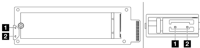
Figure 15. Voyants de l'interposeur M.2
