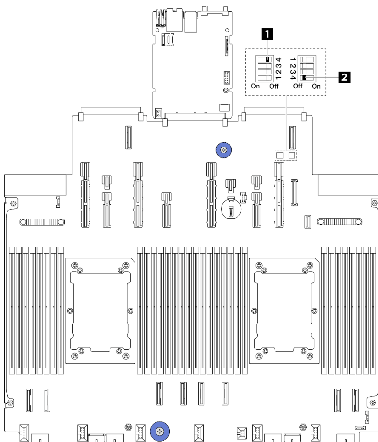
Figure 6. Commutateurs du bloc carte mère
