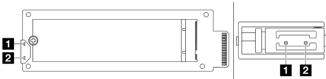
그림 15. M.2 인터포저 LED
