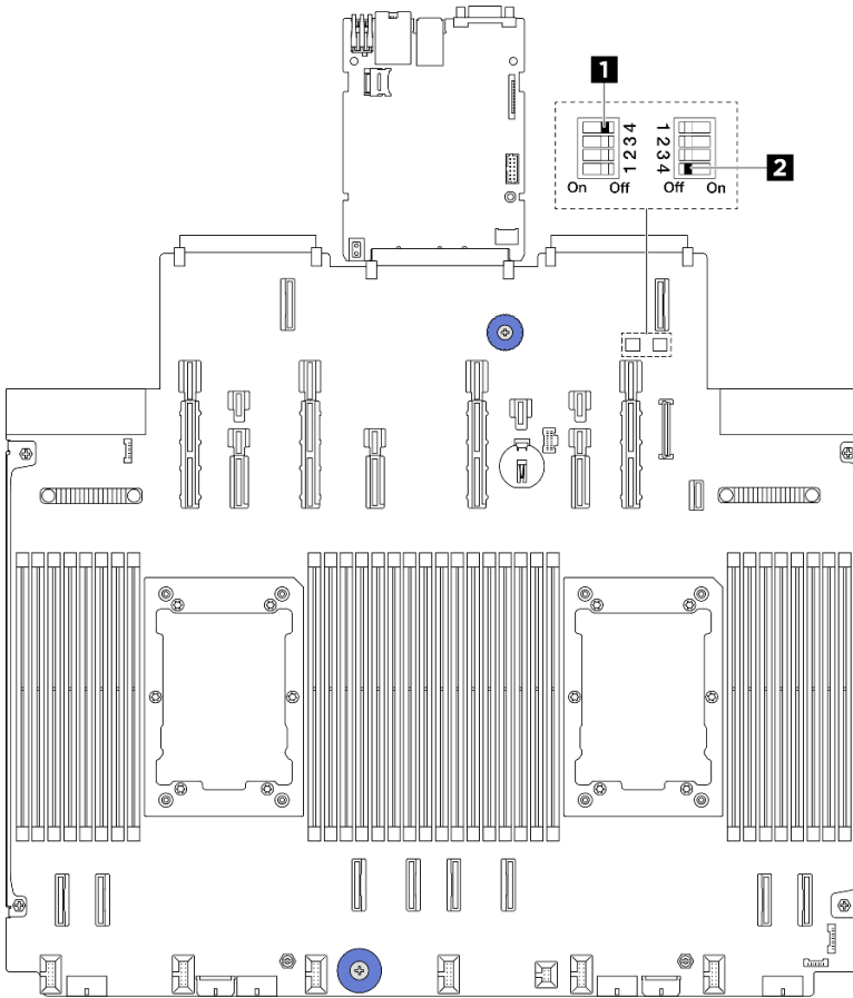
그림 6. 시스템 보드 어셈블리 스위치
