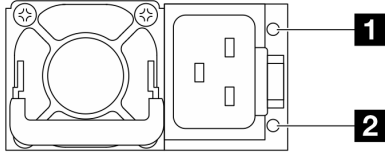
그림 12. CRPS Premium 전원 공급 장치의 LED
