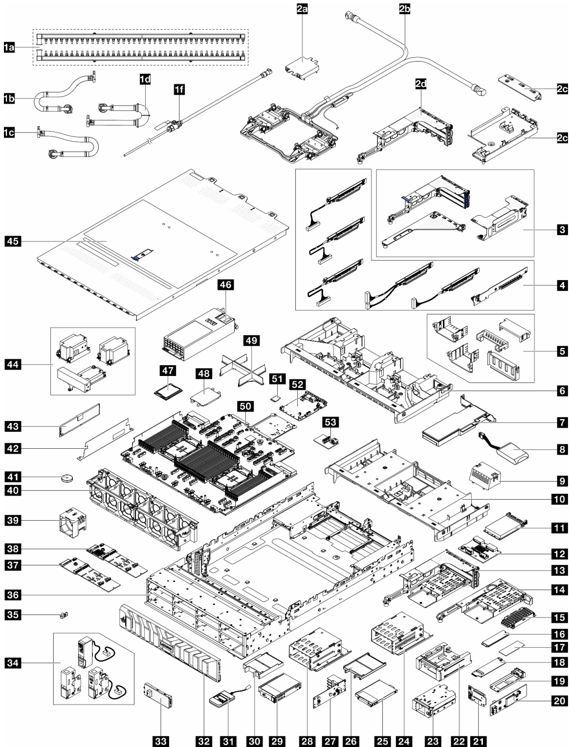
그림 21. 서버 구성 요소(E3, S 베이 새시)
