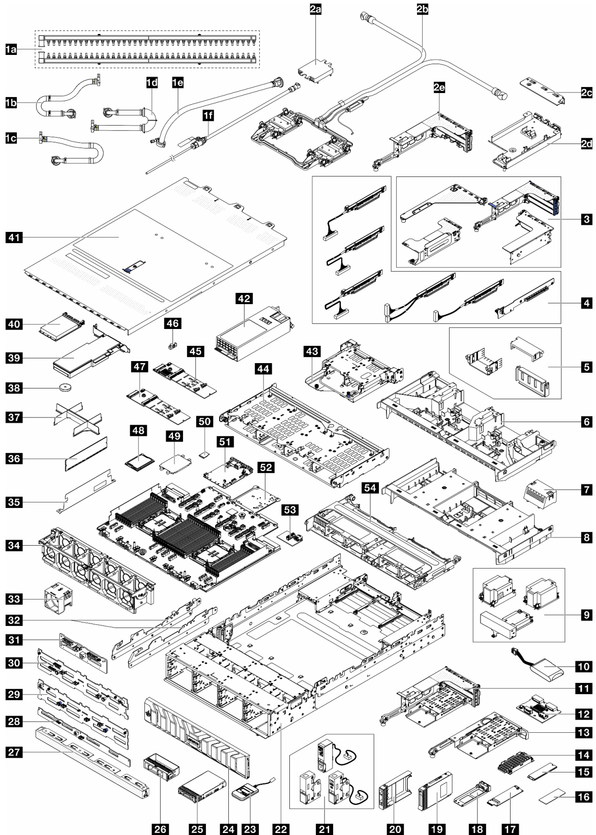
그림 20. 서버 구성 요소(3.5" 드라이브 베이 새시)
