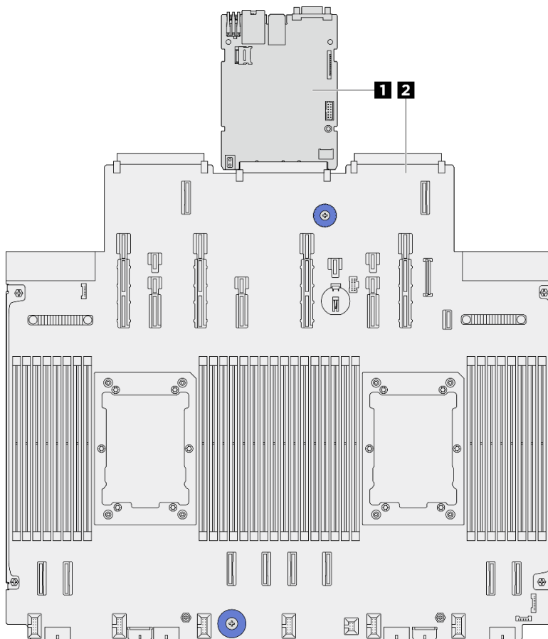
그림 4. 시스템 보드 어셈블리 레이아웃
