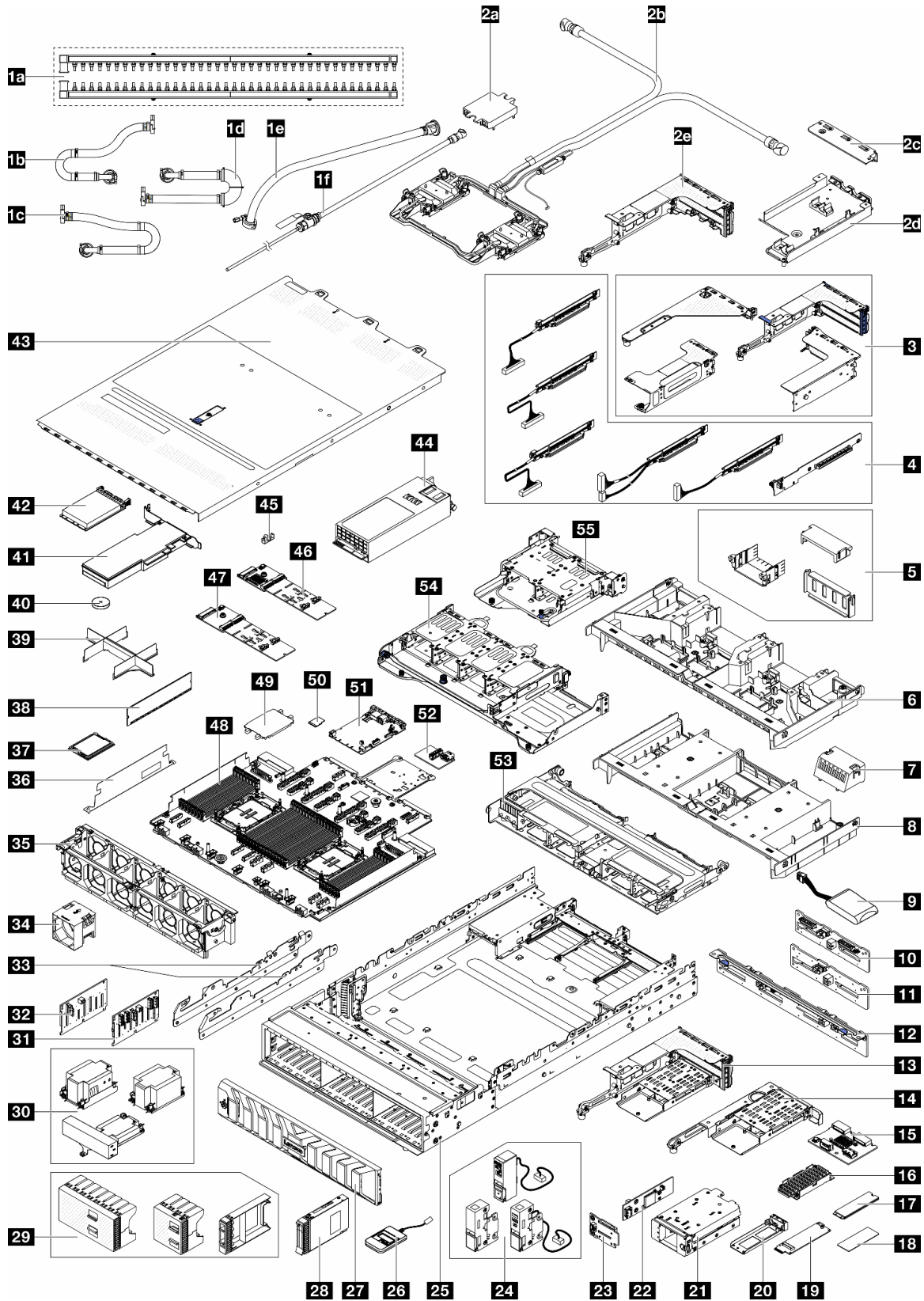
그림 19. 서버 구성 요소(2.5" 드라이브 베이 새시)
