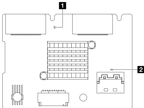
그림 16. 뒷면 M.2 백플레인 LED
