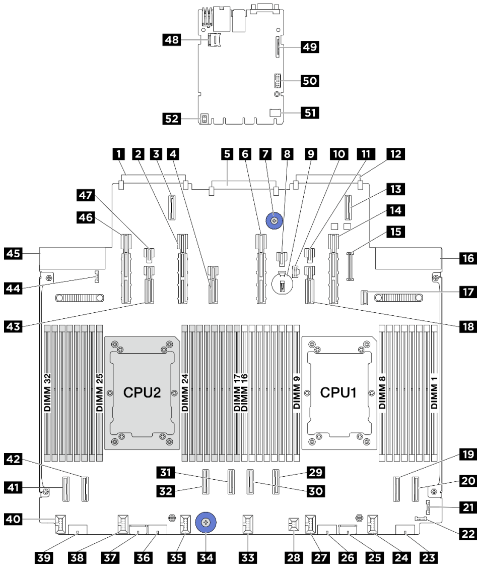
그림 5. 시스템 보드 어셈블리 커넥터
