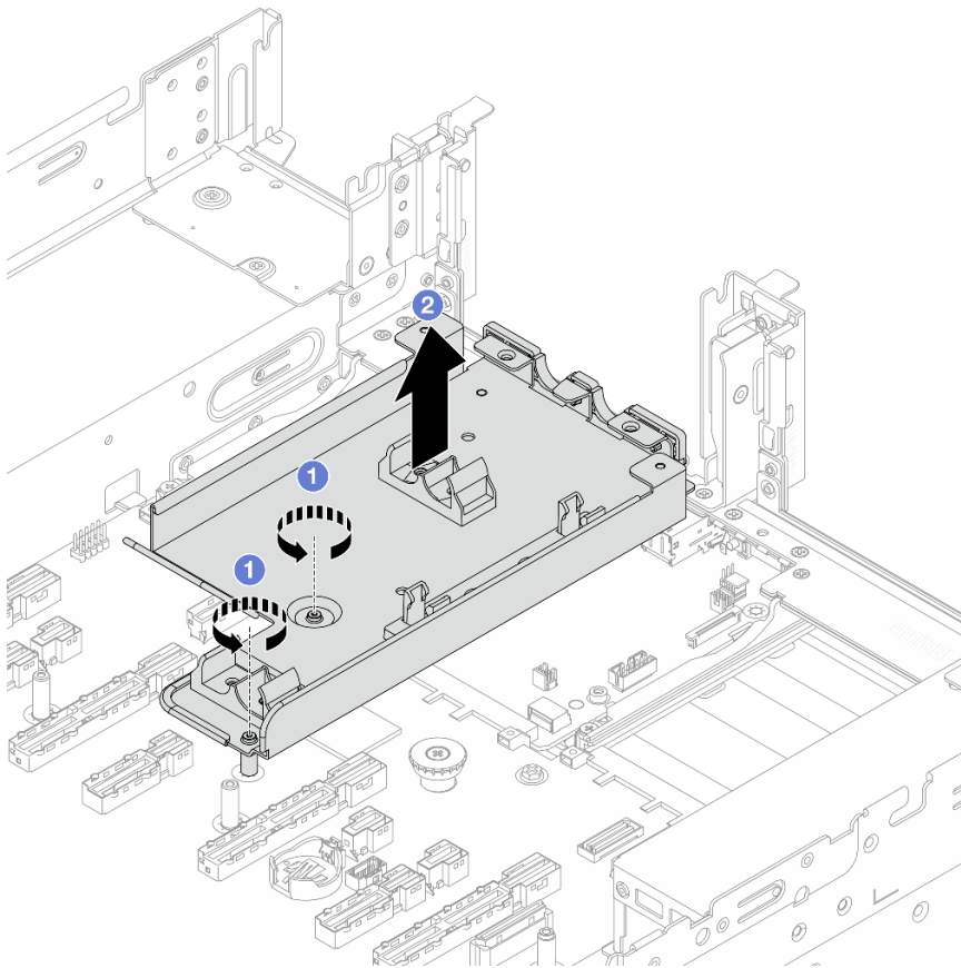
圖例 107. 卸下水管固定器
