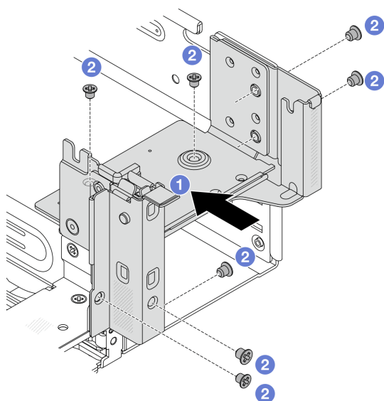
圖例 252. 安裝右側後壁托架
