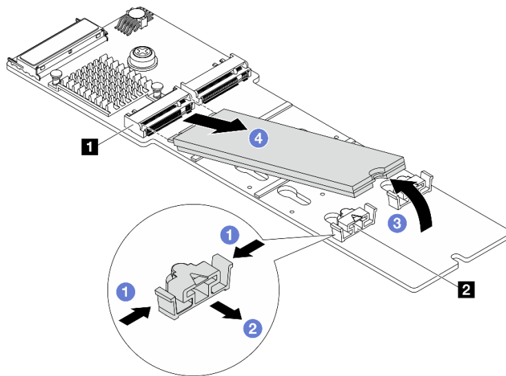
圖例 88. 卸下 M.2 硬碟
