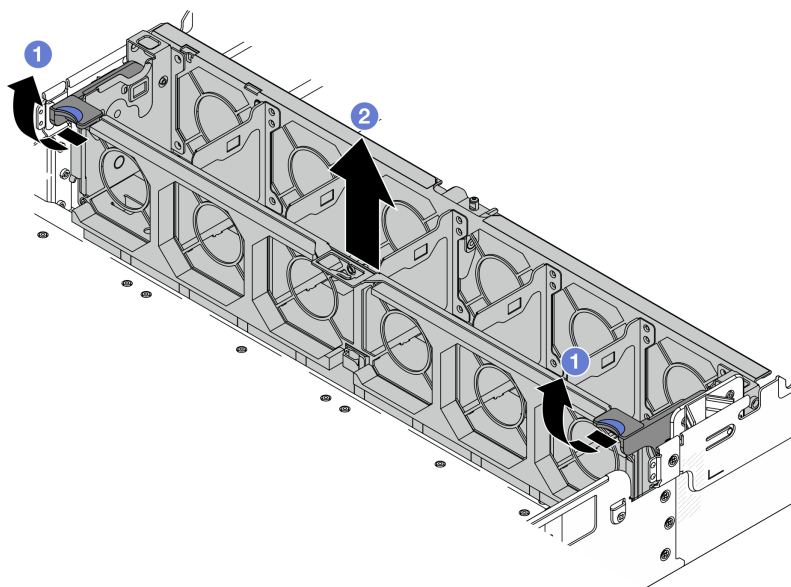
圖例 312. 卸下系統風扇機盒
