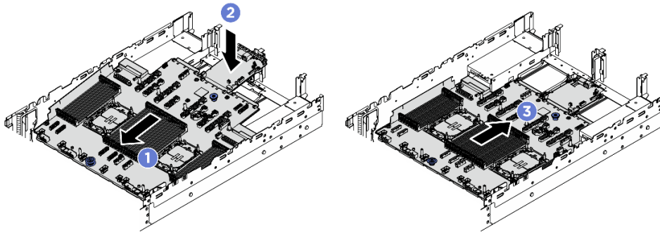
圖例 305. 安裝主機板組件
