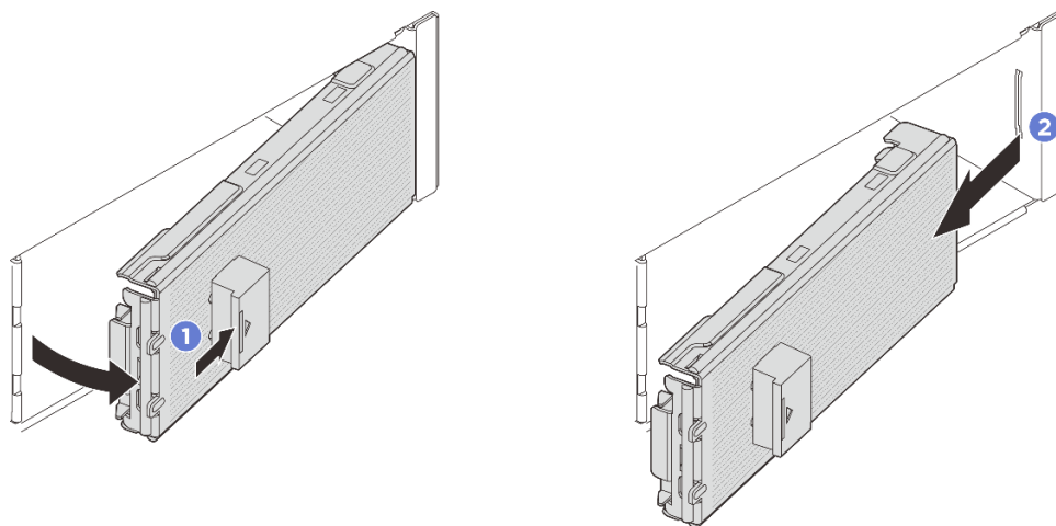
圖例 51. 卸下 E3.S 擋板
