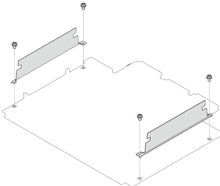
圖例 47. 卸下纜線壁
