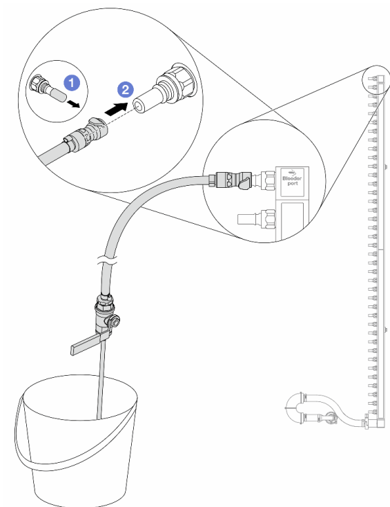
圖例 164. 在回流側安裝洩放套件
