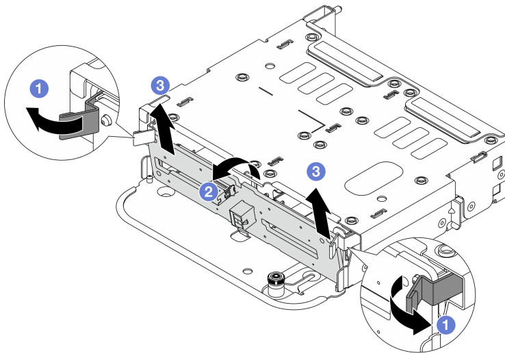
圖例 253. 卸下後方 4 x 2.5 吋後方硬碟背板
