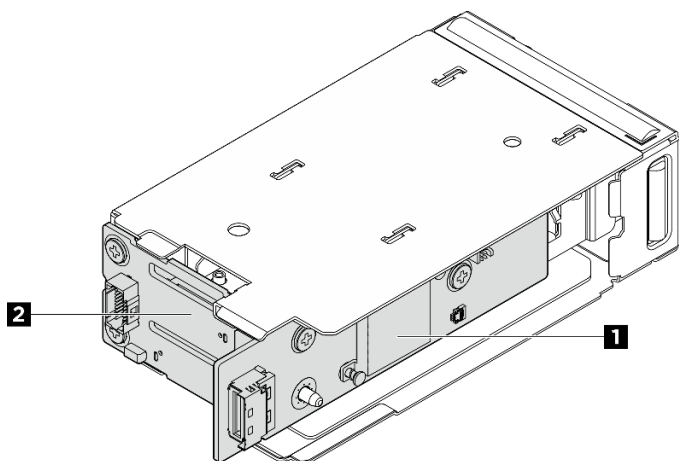
圖例 138. 前方 M.2 硬碟背板
