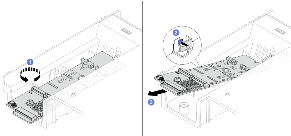
圖例 93. 從空氣擋板卸下 M.2 背板
