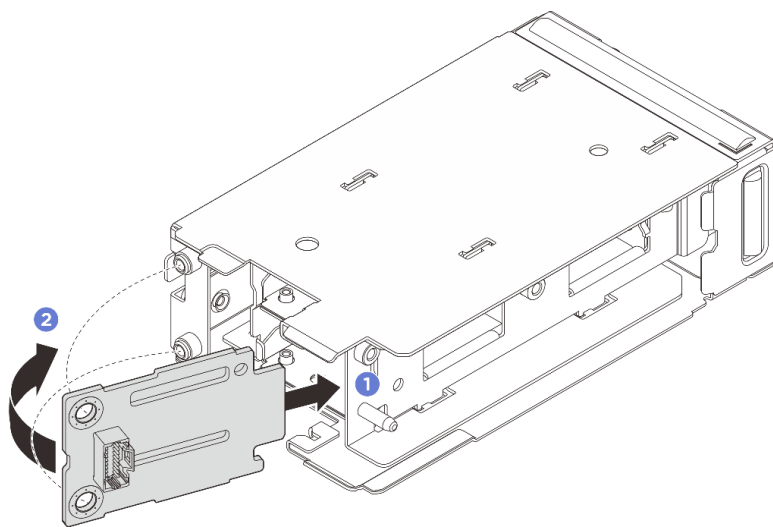
圖例 139. 安裝 M.2 開機背板
