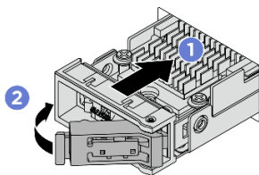
圖例 122. 安裝 M.2 硬碟組件
