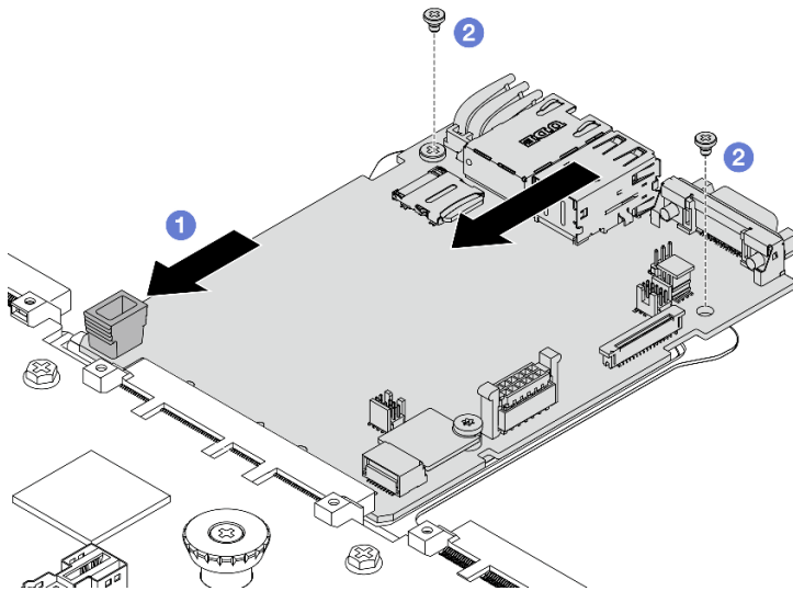
圖例 308. 將系統 I/O 板安裝在處理器板上
