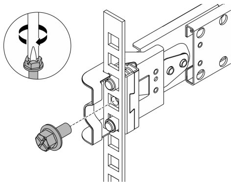
圖例 28. 將伺服器固定到機架背面
