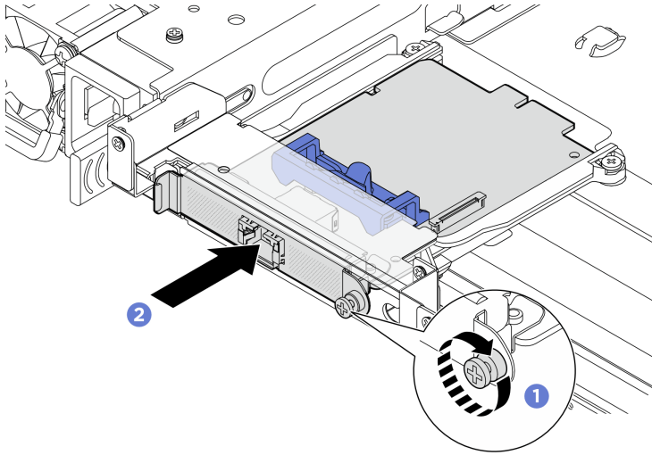
圖例 151. 安裝管理 NIC 配接卡
