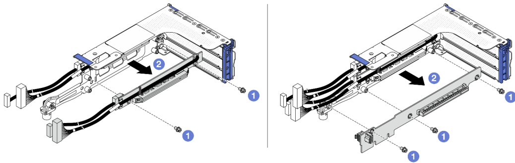
圖例 282. 從擴充卡匣卸下擴充卡
