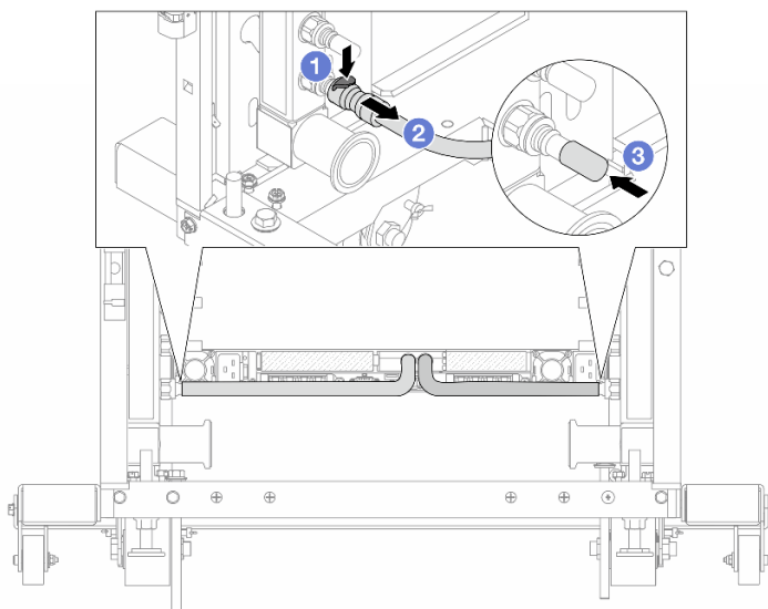
圖例 159. 卸下快速連接插頭
