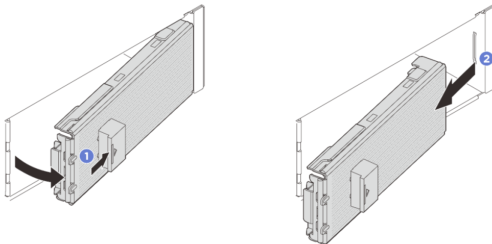
圖例 66. 卸下 E3.S 擋板
