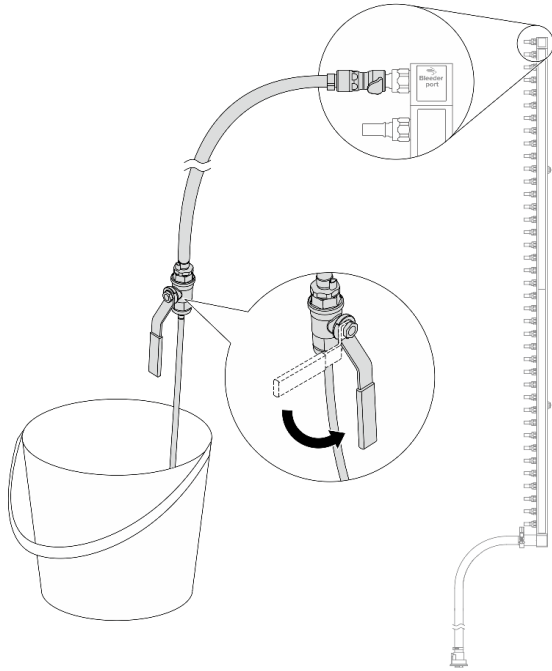
圖例 187. 開啟洩放閥門
