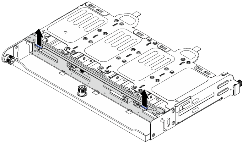
圖例 254. 卸下後方 8 x 2.5 吋後方硬碟背板
