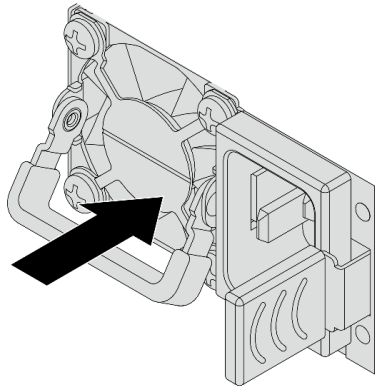
圖例 215. 安裝熱抽換電源供應器
