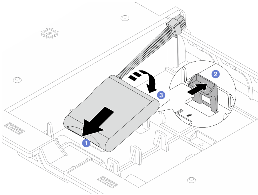
圖例 240. 將 RAID 快閃記憶體電源模組安裝在空氣擋板上
