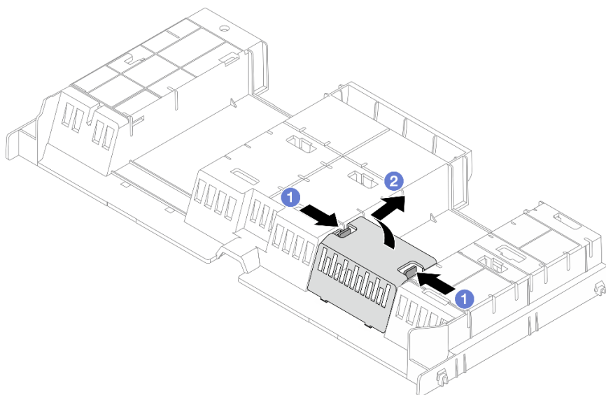
圖例 43. 卸下空氣擋板填充板
