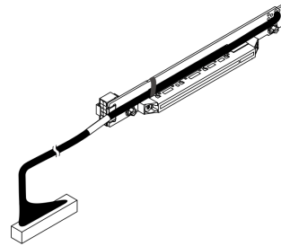
圖例 9. 含電源接頭的含纜線擴充卡 ( Gen5 x16 , 300 公釐 , 插槽 3/6 )
