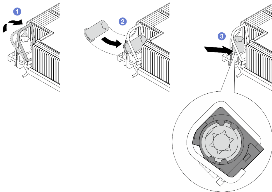
圖例 85. 將 Torx T30 螺帽安裝到散熱槽
