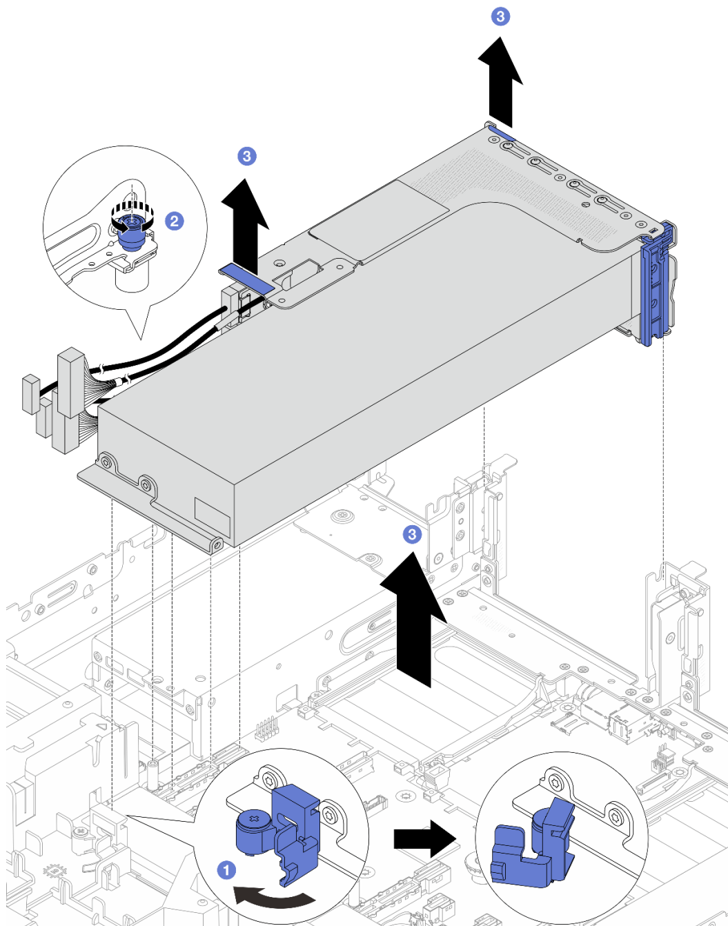
圖例 80. 卸下擴充卡組件
