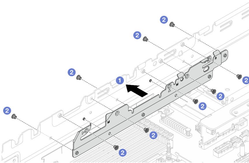
圖例 206. 安裝中間托架
