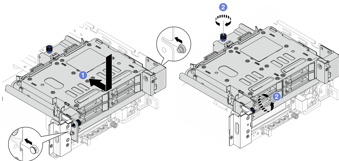
圖例 261. 安裝 4 x 2.5 吋背面框架
