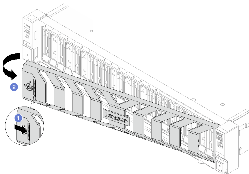
圖例 291. 卸下安全擋板
