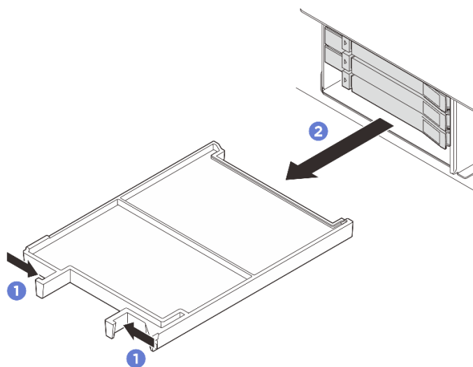
圖例 67. 卸下機槽填充板
