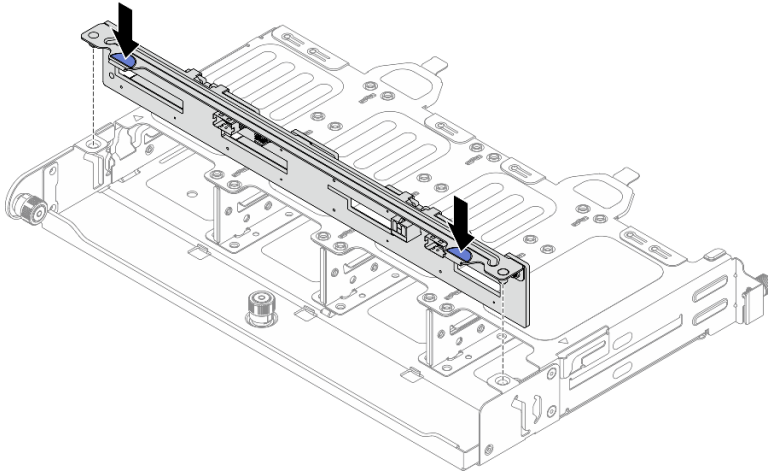
圖例 257. 安裝 8 x 2.5 吋後方硬碟背板
