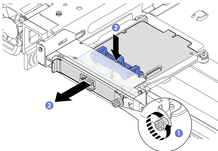
圖例 150. 卸下管理 NIC 配接卡
