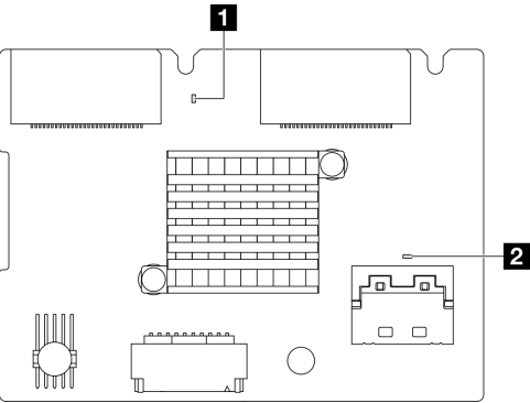
圖例 330. 背面 M.2 背板 LED
