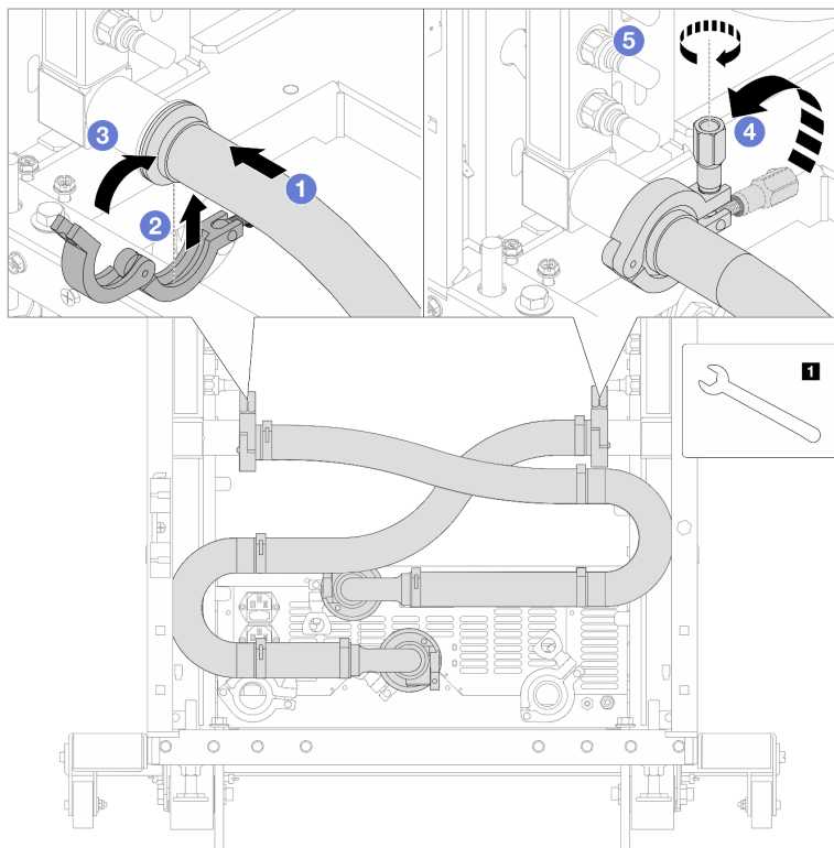
圖例 170. 安裝連接套組
