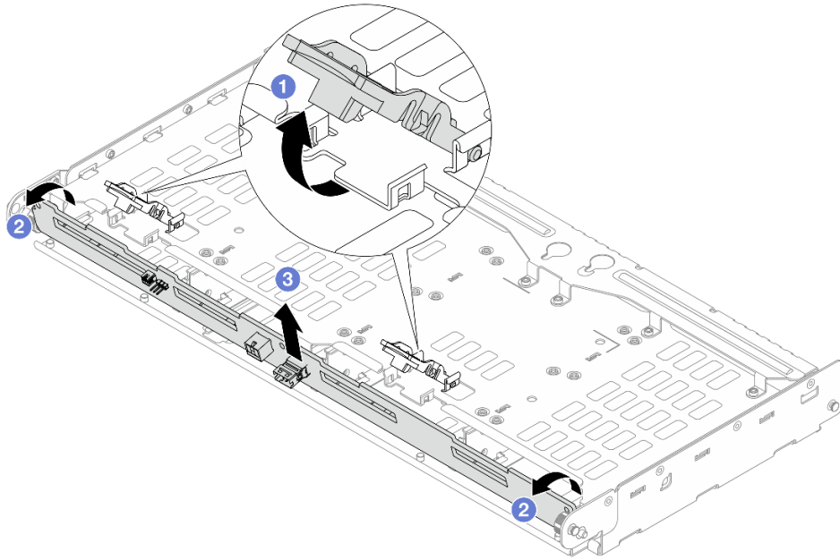
圖例 255. 卸下後方 4 x 3.5 吋後方硬碟背板
