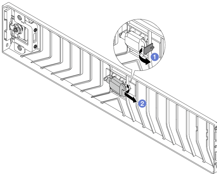
圖例 292. 取出鑰匙
