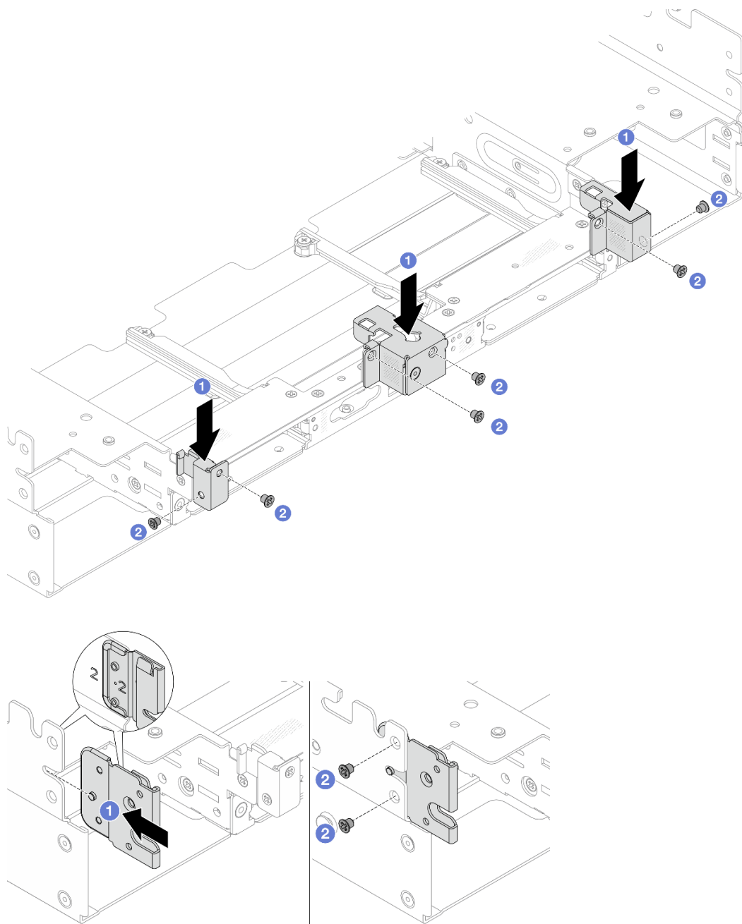
圖例 268. 安裝 4 x 3.5 吋後方框架組件的後壁托架
