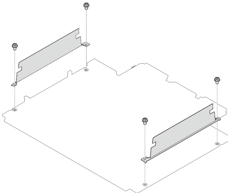
圖例 48. 安裝纜線壁
