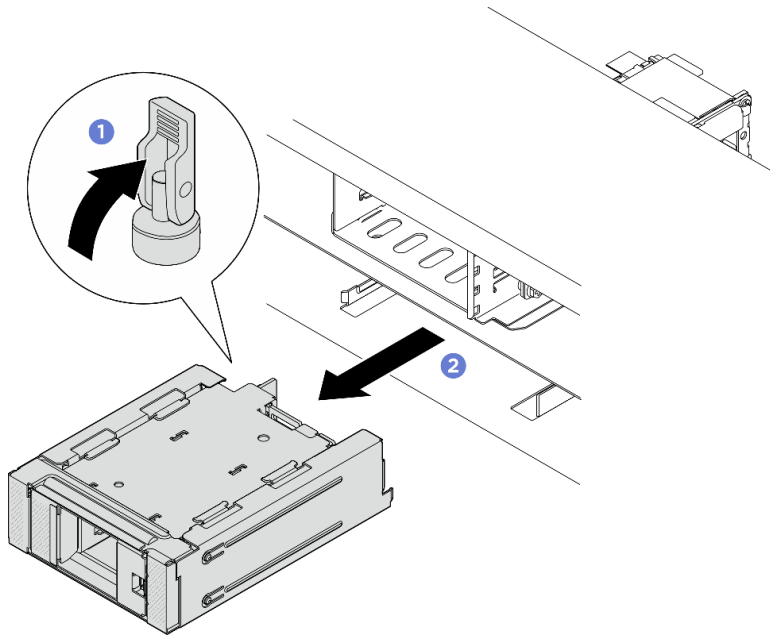
圖例 132. 卸下前方 M.2 框架及其機架
