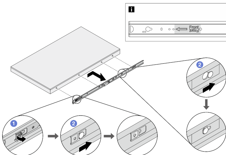
圖例 22. 卸下內滑軌
