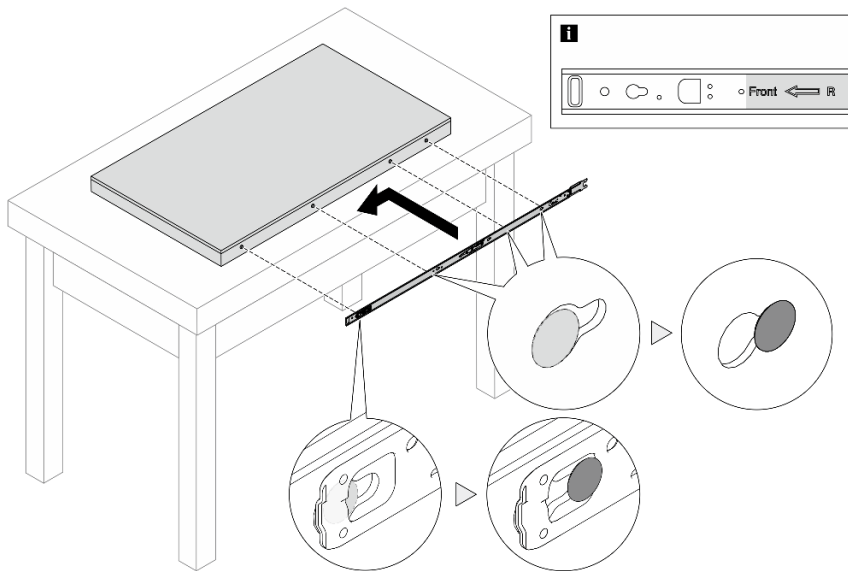
圖例 34. 安裝內滑軌
