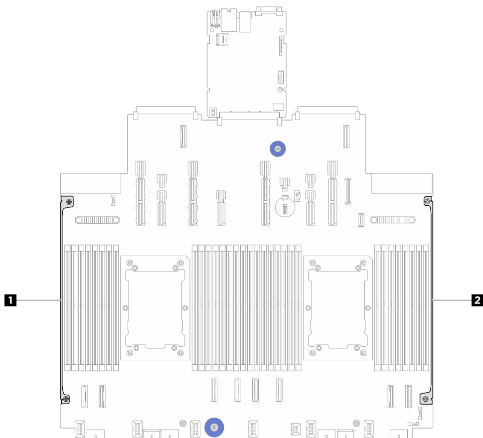
圖例 46. 纜線壁位置
