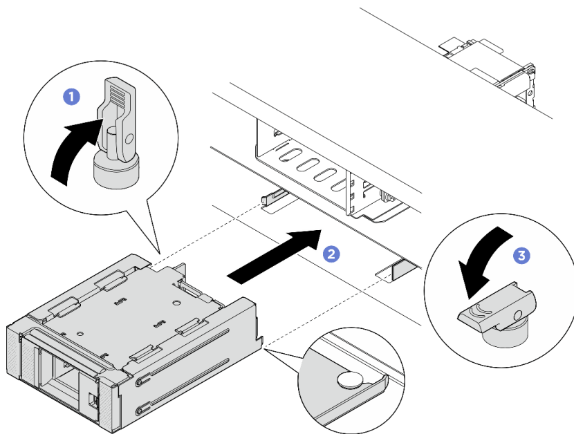
圖例 144. 安裝前方 M.2 框架及其機架
