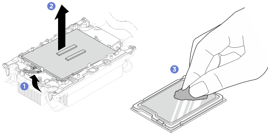
圖例 221. 將處理器與散熱槽和支架分開
