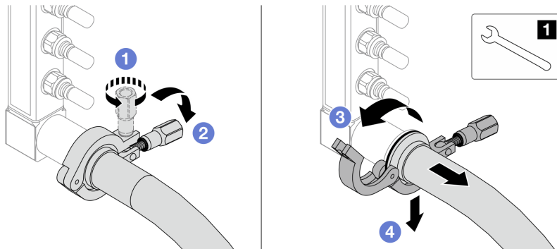
圖例 188. 將歧管與軟管套件分離
