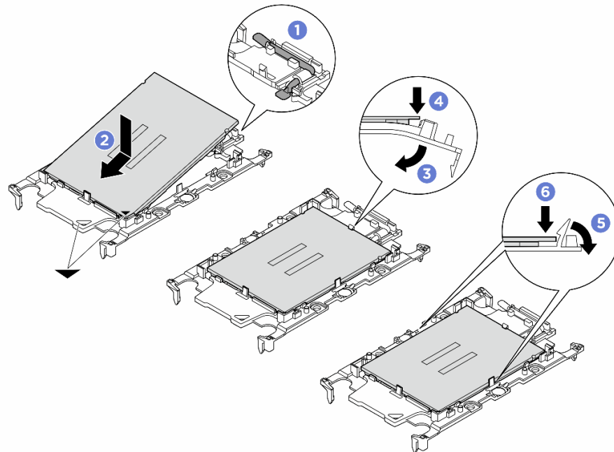
圖例 224. 安裝處理器支架
