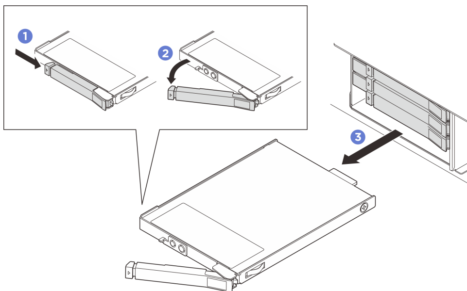
圖例 65. 卸下 E3.S 熱抽換硬碟
