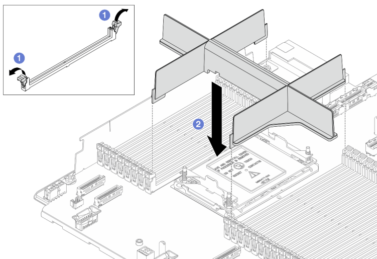
圖例 220. 安裝 PHM 填充板
