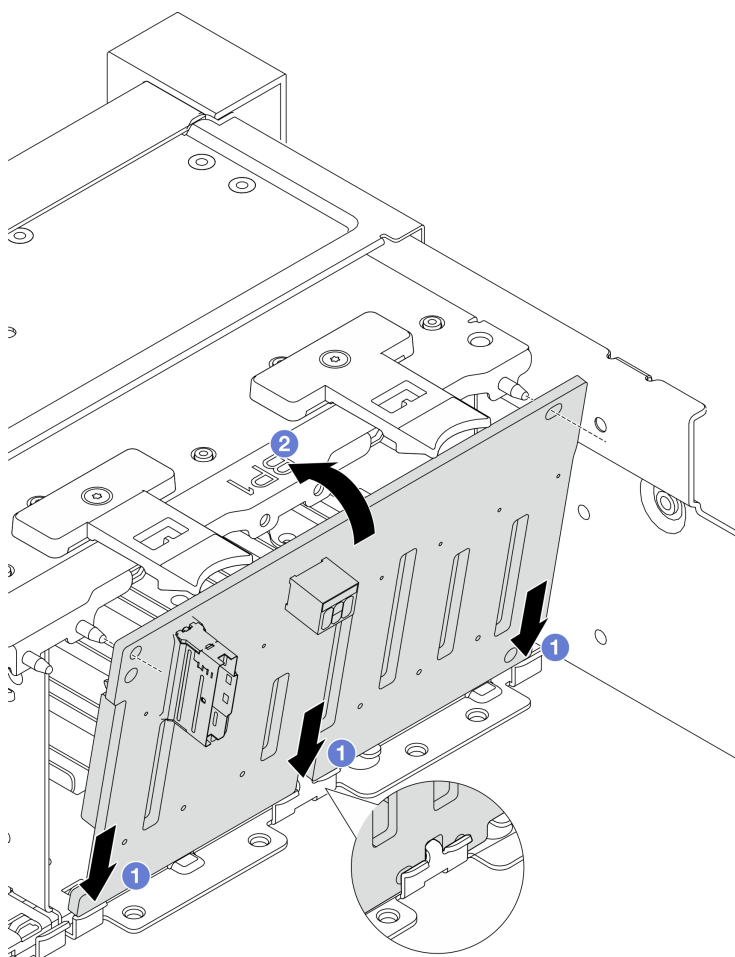
圖例 78. 安裝前方 2.5 吋硬碟背板
