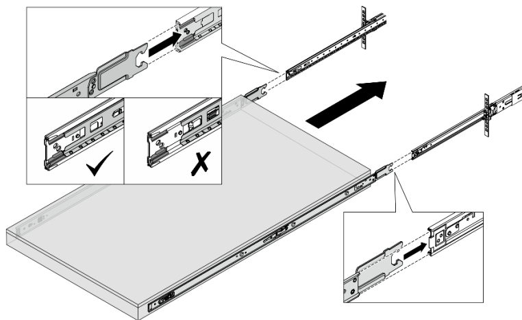
圖例 36. 交互鎖定滑軌
