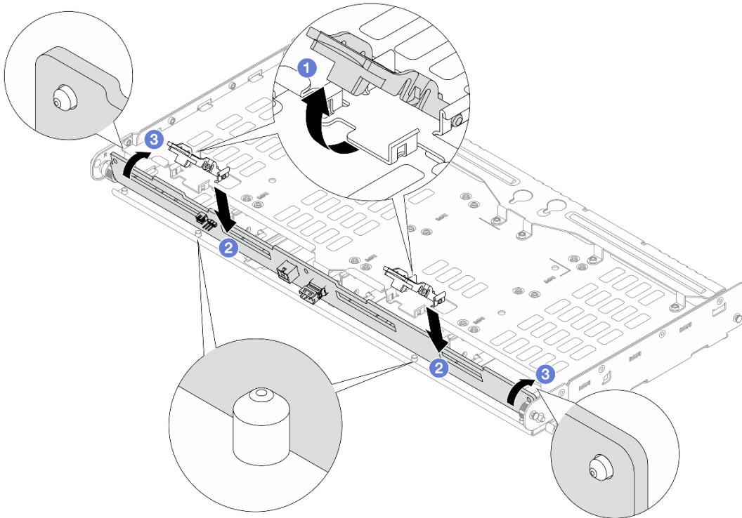
圖例 258. 安裝 4 x 3.5 吋後方硬碟背板
