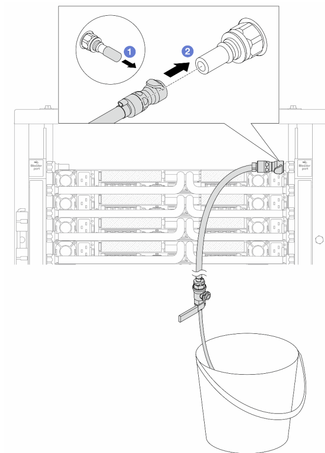
圖例 178. 在回流側安裝洩放套件
