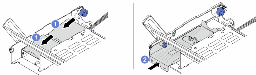
圖例 244. 將 RAID 快閃記憶體電源模組安裝在中間框架上
