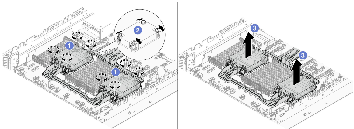
圖例 106. 卸下 Processor Neptune Core Module
