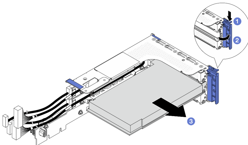
圖例 279. 從 3FH 擴充卡匣卸下 PCIe 配接卡
