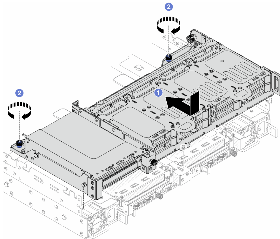
圖例 266. 安裝 8 x 2.5 吋背面框架
