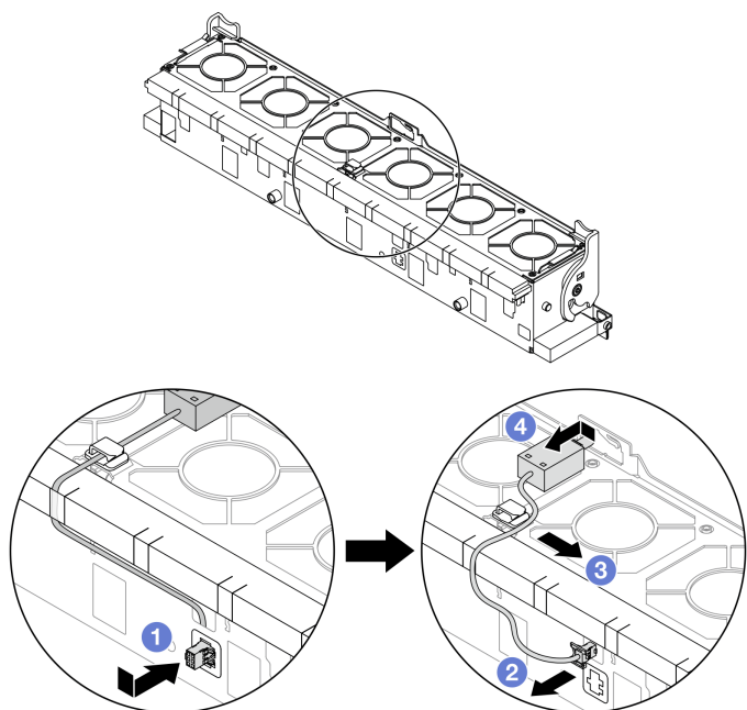
圖例 101. 卸下入侵開關
