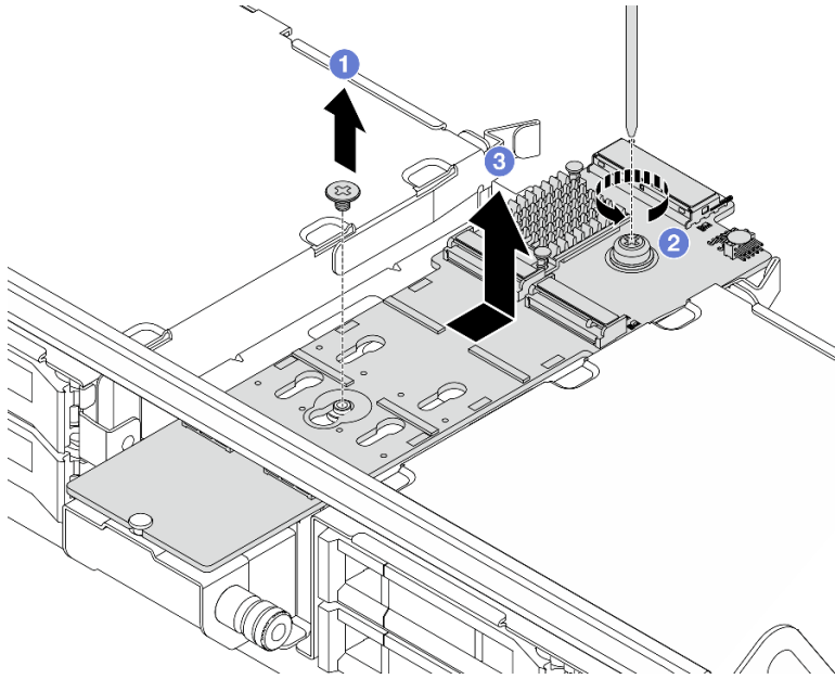
圖例 95. 從中間框架卸下 M.2 背板
