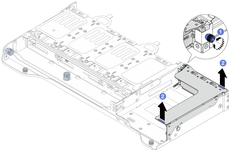
圖例 277. 卸下 2FH 擴充卡組件
