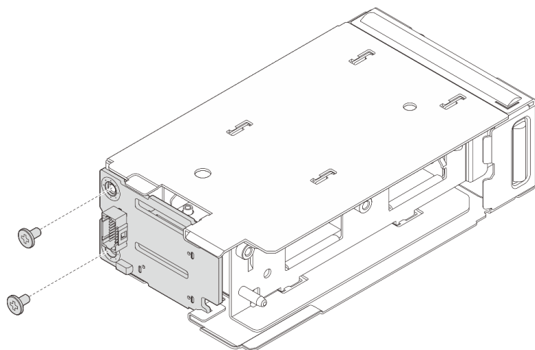
圖例 140. 安裝 M.2 開機背板
