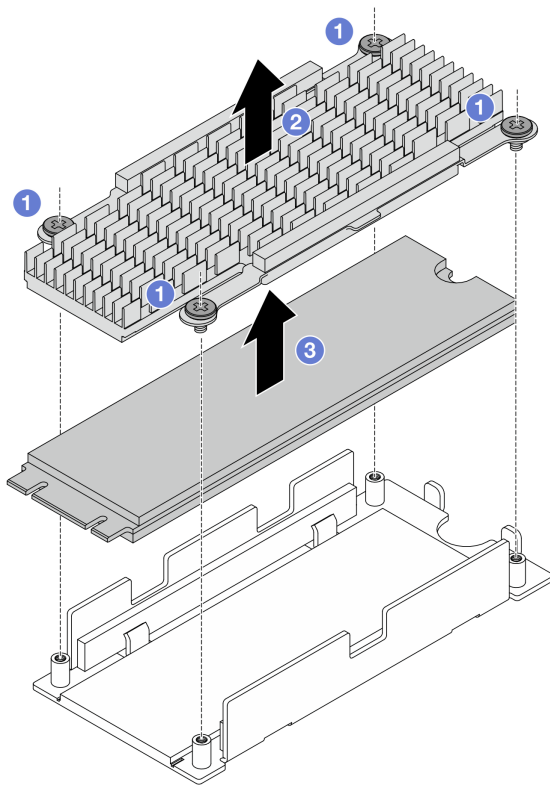
圖例 125. 卸下 M.2 硬碟
