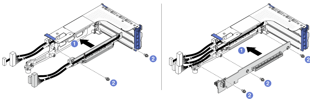
圖例 283. 在 3FH 擴充卡匣上安裝擴充卡
