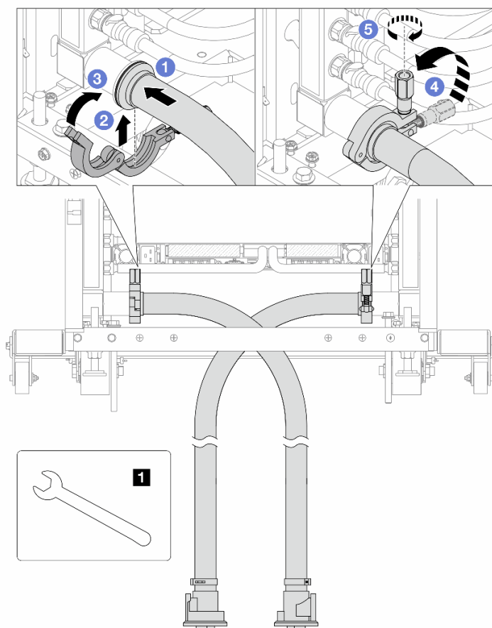
圖例 191. 安裝水管套件
