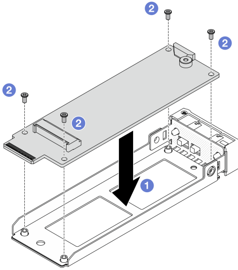
圖例 129. 安裝 M.2 轉插卡
