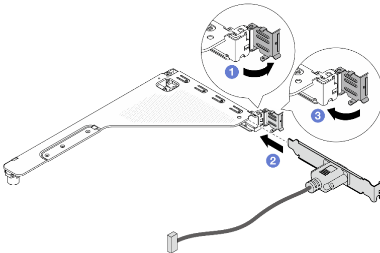
圖例 299. 安裝序列埠模組
