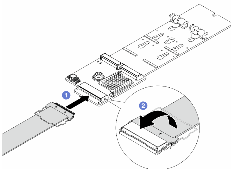
圖例 99. 連接 M.2 纜線
