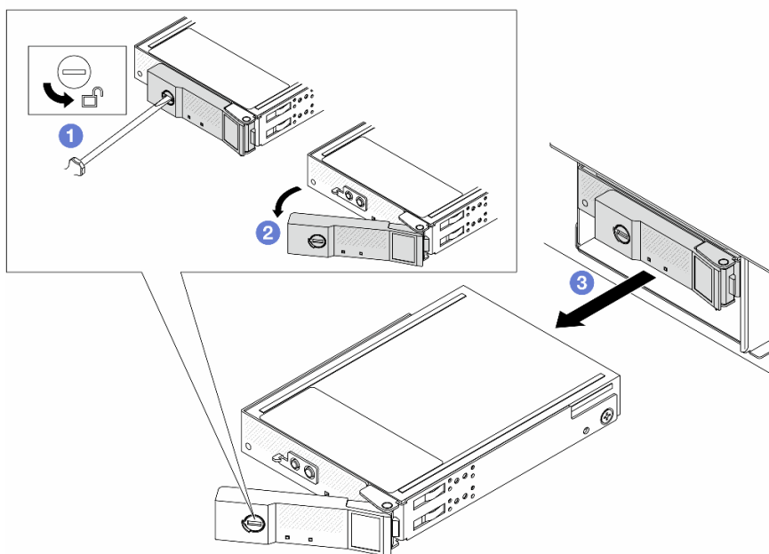
圖例 52. 卸下 CMM
