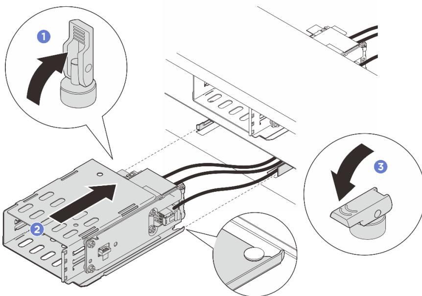
圖例 75. 安裝 E3.S 1T 框架
