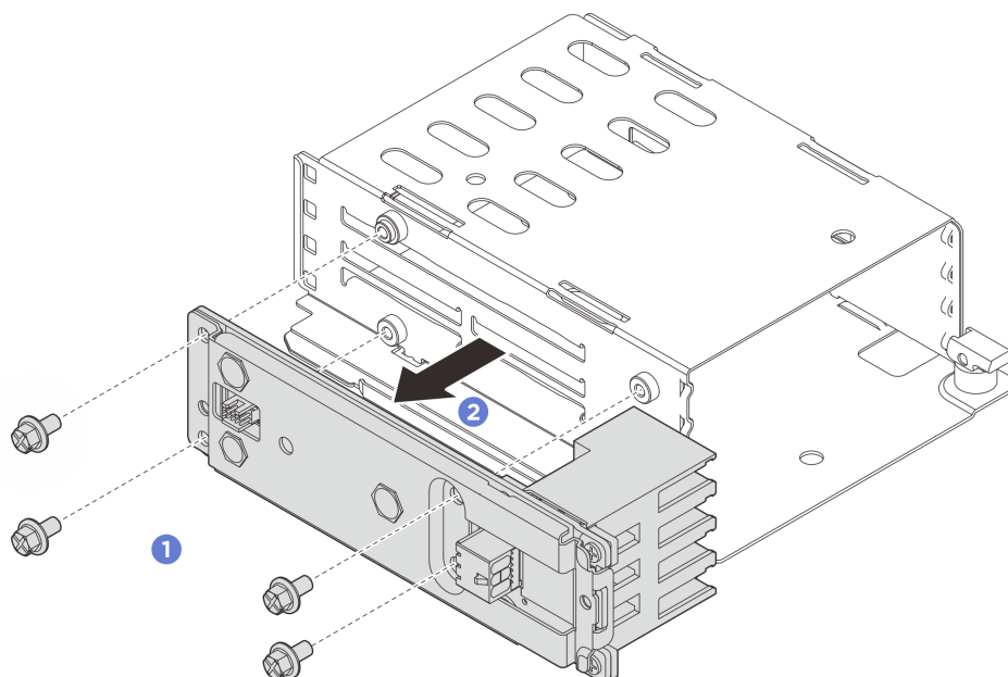
圖例 73. 卸下背板組件
