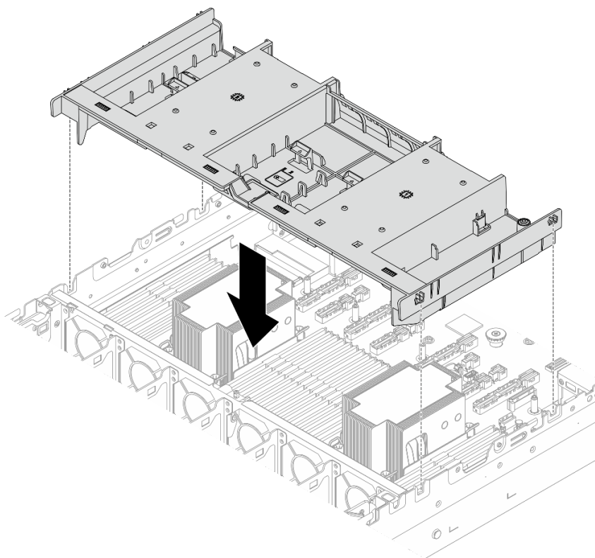
圖例 45. 安裝空氣擋板
