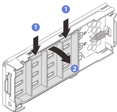
圖例 70. 卸下內板
