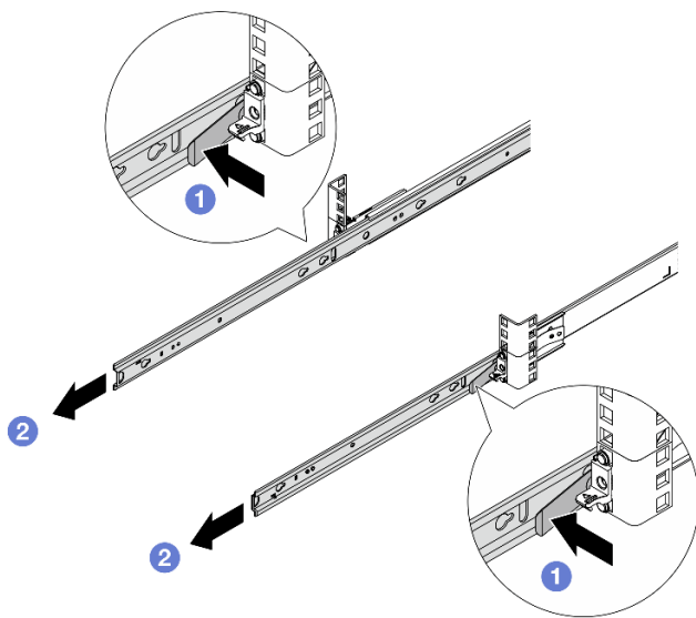
圖例 23. 卸下內滑軌
