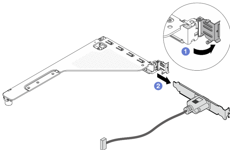
圖例 296. 卸下序列埠模組
