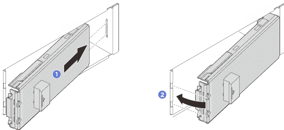
圖例 71. 安裝 E3.S 擋板
