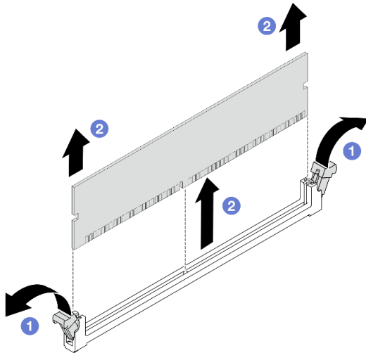
圖例 200. 卸下記憶體模組
