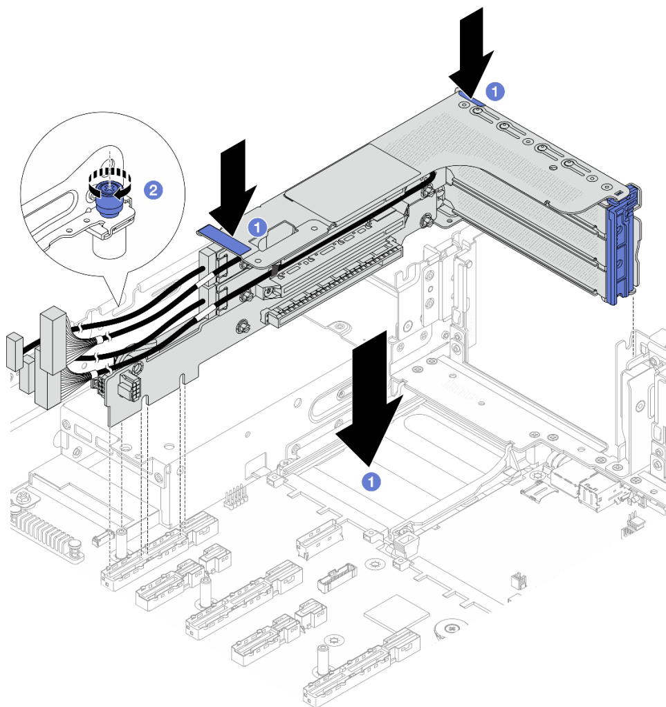
圖例 288. 安裝 3FH 擴充卡組件
