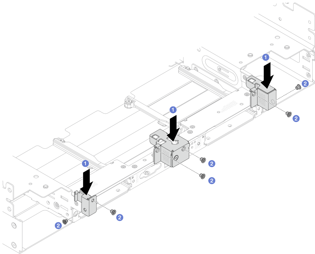
圖例 264. 安裝 8 x 2.5 吋後方框架組件的後壁托架
