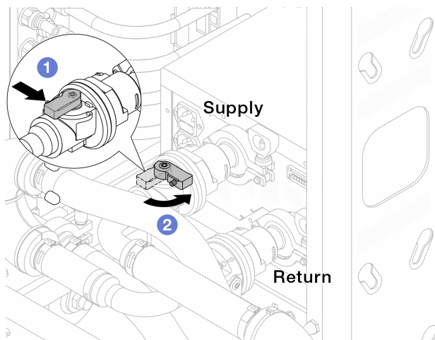
圖例 158. 關閉球閥
