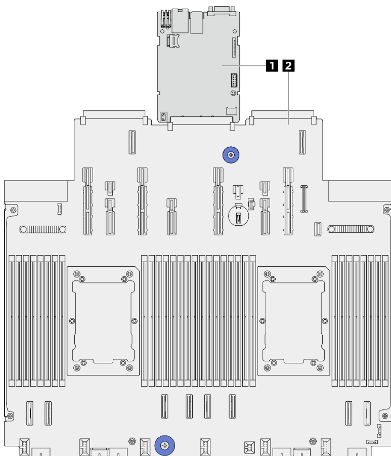
圖例 301. 主機板組件佈置
