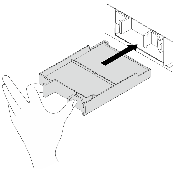
圖例 53. 安裝 CMM 機槽填充板
