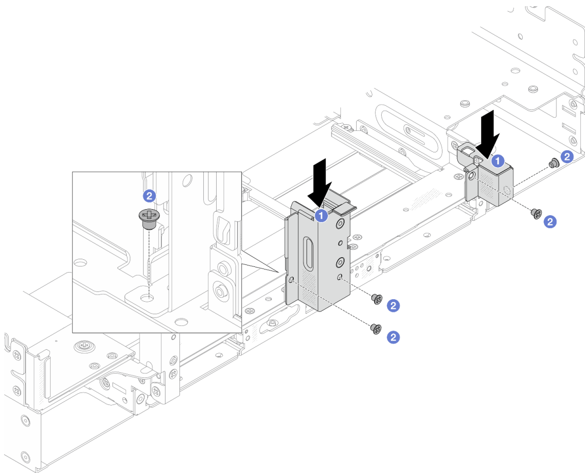
圖例 260. 安裝 4 x 2.5 吋背面框架的後壁托架
