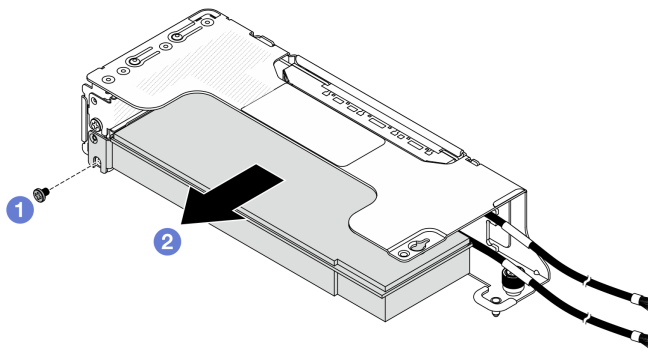
圖例 278. 從 2LP 擴充卡匣卸下 PCIe 配接卡
