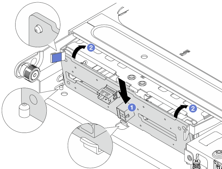
圖例 207. 安裝 2.5 吋中間硬碟背板
