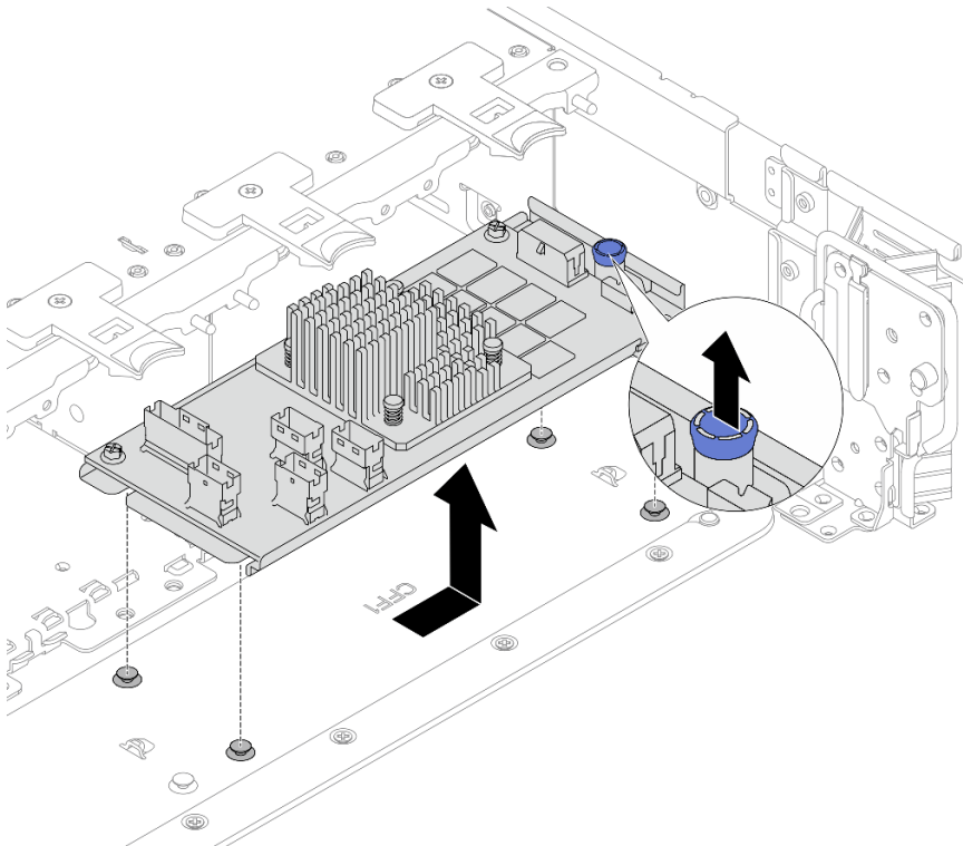
圖例 86. 卸下內部 CFF 配接卡
