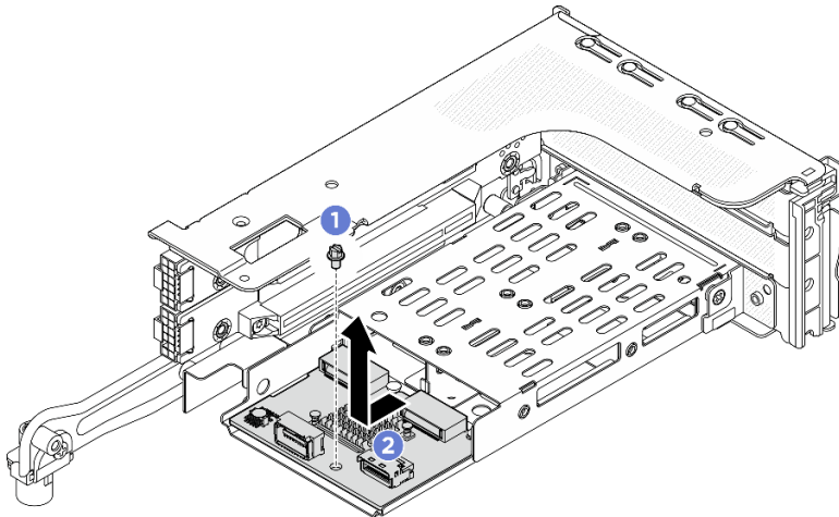
圖例 146. 從 3FH M.2 擴充卡匣中卸下 M.2 背板
