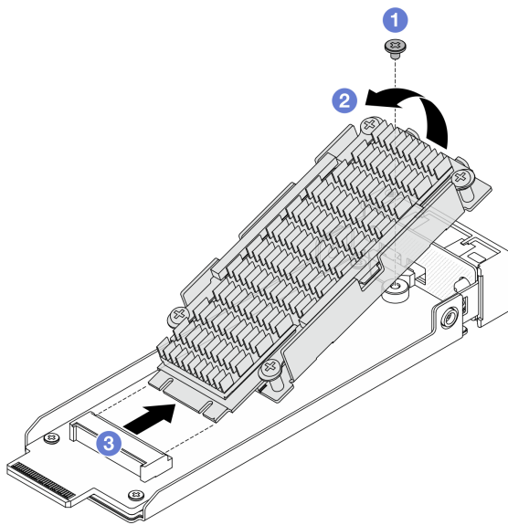
圖例 123. 卸下帶有散熱槽的 M.2 硬碟
