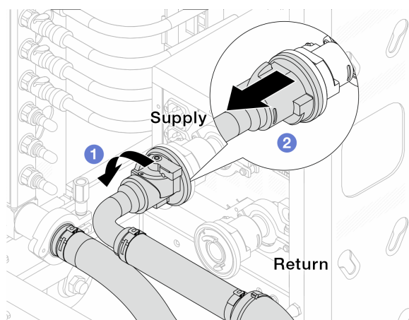
圖例 160. 卸下連接套組
