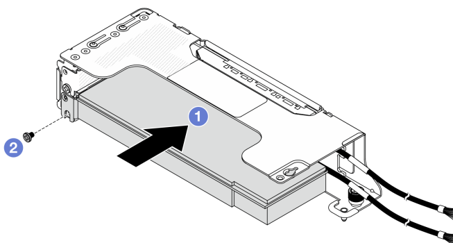
圖例 284. 在 2LP 擴充卡匣上安裝 PCIe 配接卡
