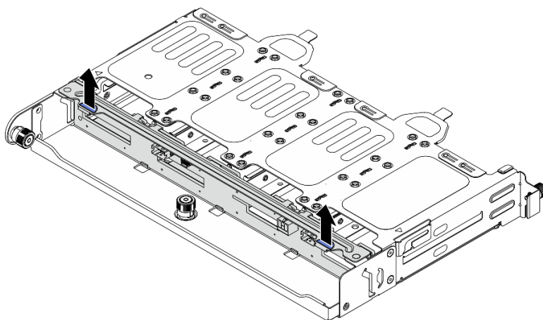
圖例 263. 卸下後方 8 x 2.5 吋後方硬碟背板
