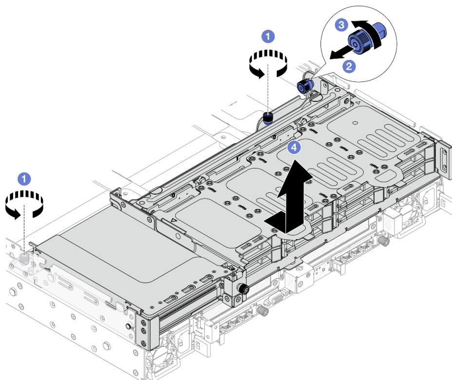
圖例 262. 卸下 8 x 2.5 吋背面框架
