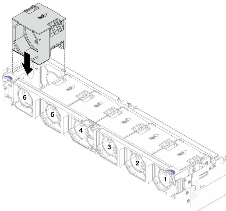
圖例 311. 安裝系統風扇
