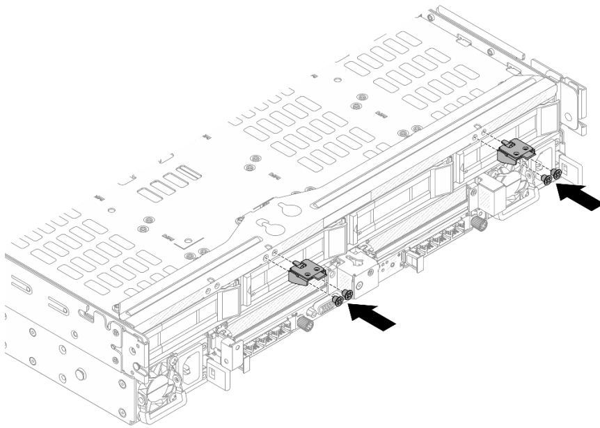
圖例 271. 安裝上蓋支撐托架
