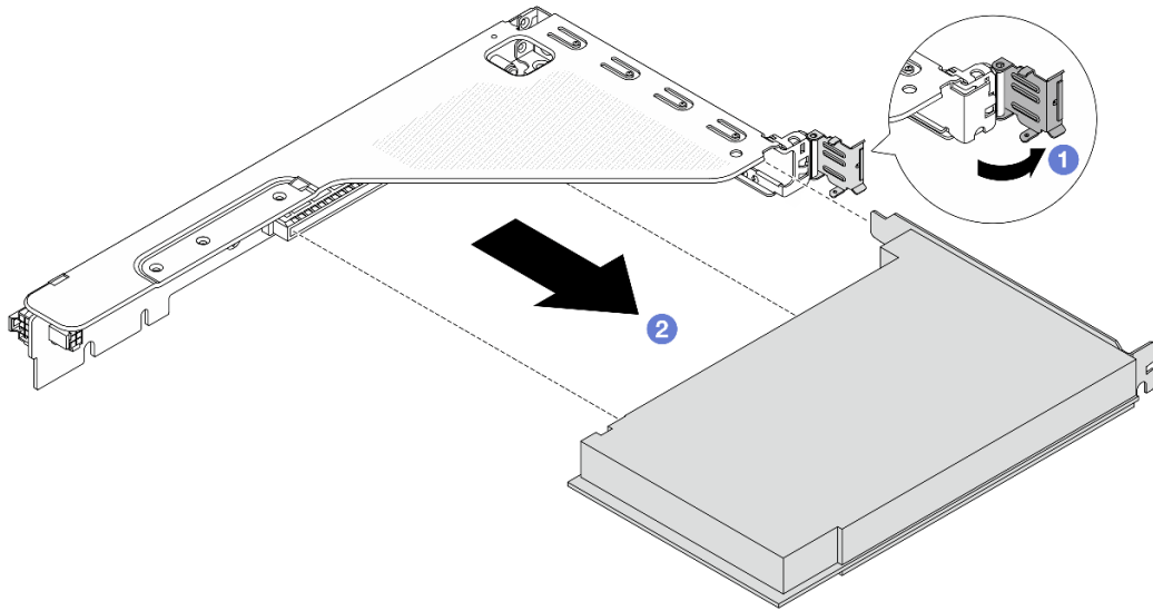
圖例 281. 從 1FH 擴充卡匣卸下 PCIe 配接卡
