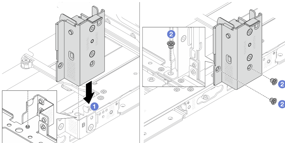
圖例 251. 安裝中間後壁托架
