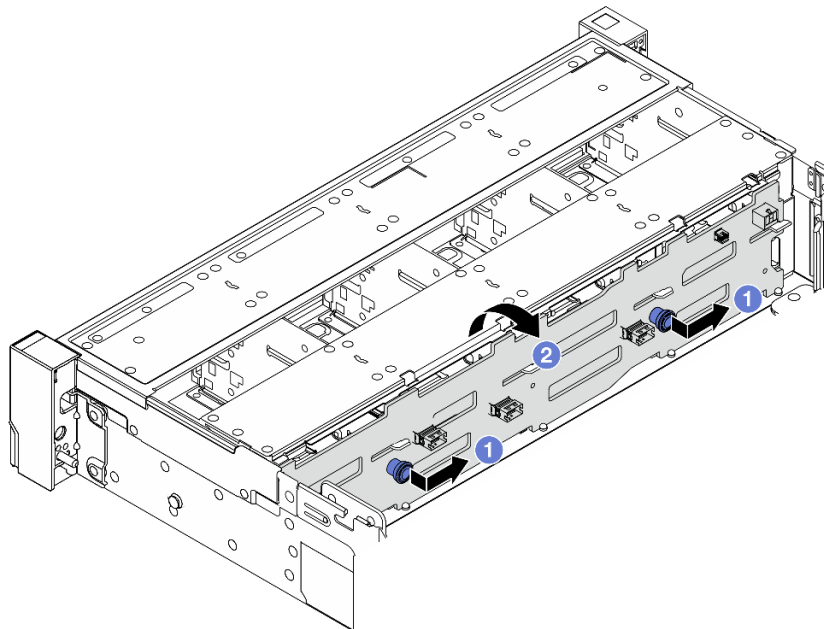
圖例 77. 卸下前方 3.5 吋硬碟背板
