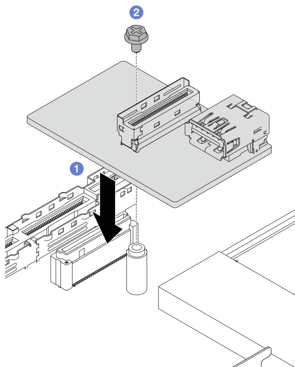
圖例 317. 安裝 USB I/O 板
