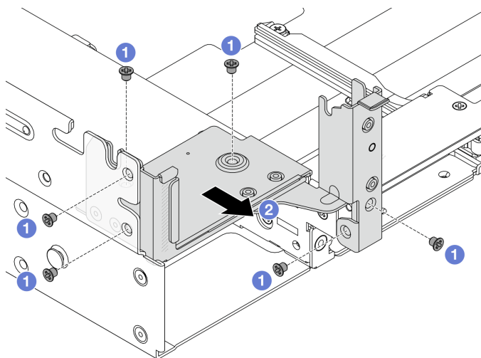
圖例 247. 卸下左側後壁托架
