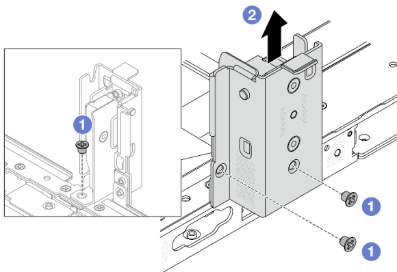
圖例 248. 卸下中間後壁托架
