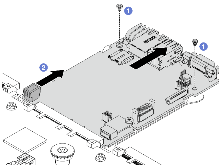
圖例 303. 將系統 I/O 板與處理器板分開
