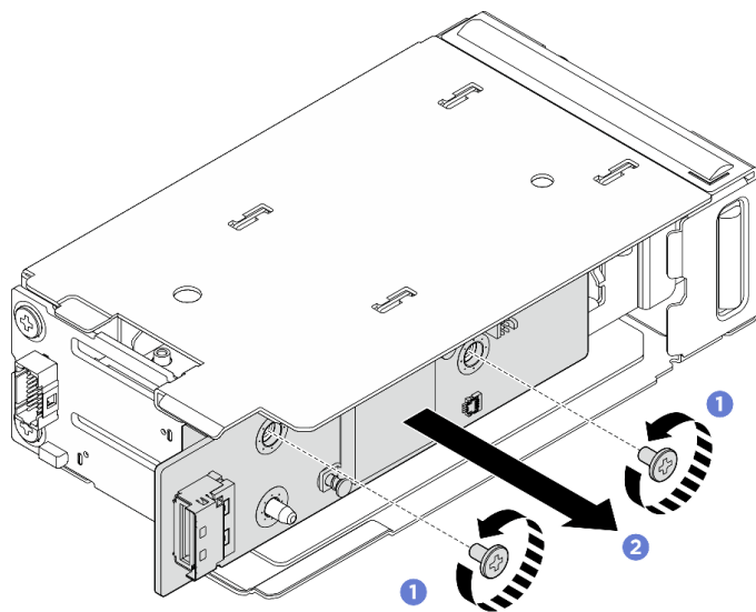
圖例 135. 卸下前方 M.2 控制器板
