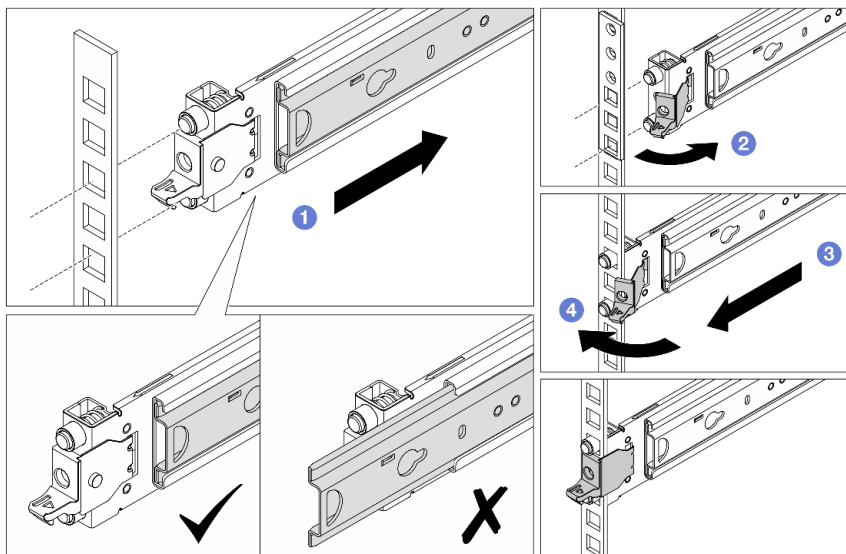
圖例 16. 安裝前方安裝插腳
