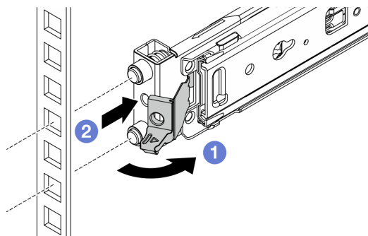
圖例 13. 從前方卸下滑軌
