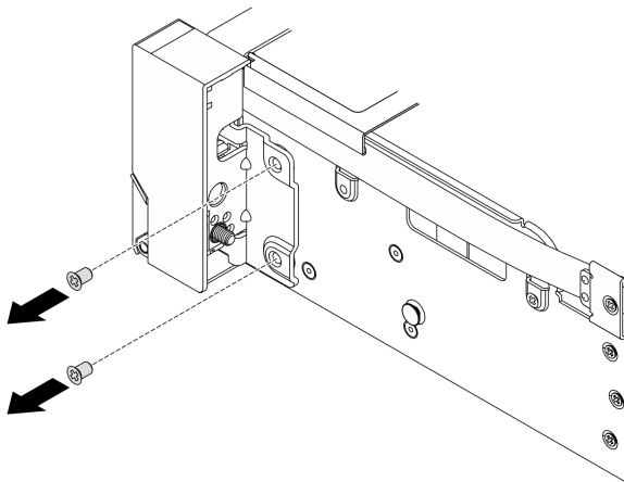
圖例 231. 卸下螺絲
