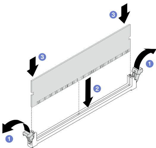
圖例 201. 安裝記憶體模組
