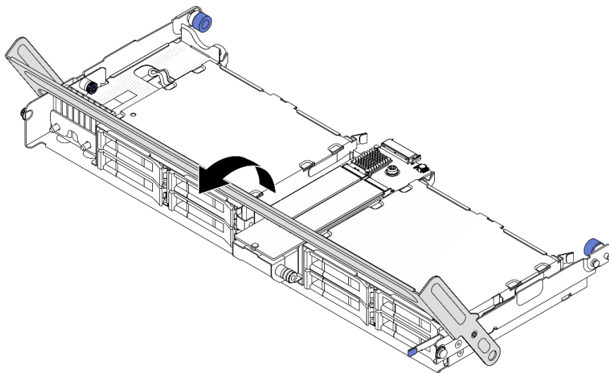
圖例 94. 打開中間框架的把手
