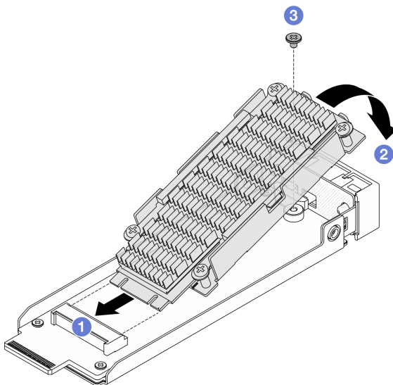
圖例 130. 安裝帶散熱槽的 M.2 硬碟
