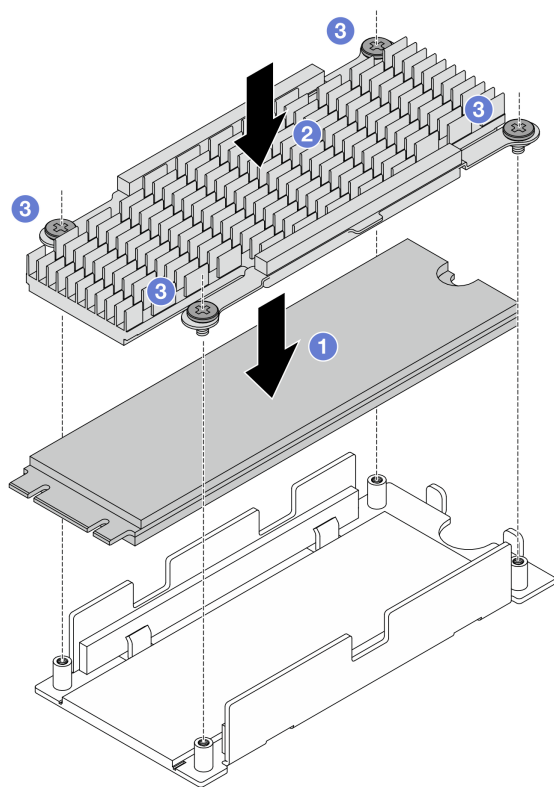
圖例 128. 安裝 M.2 硬碟
