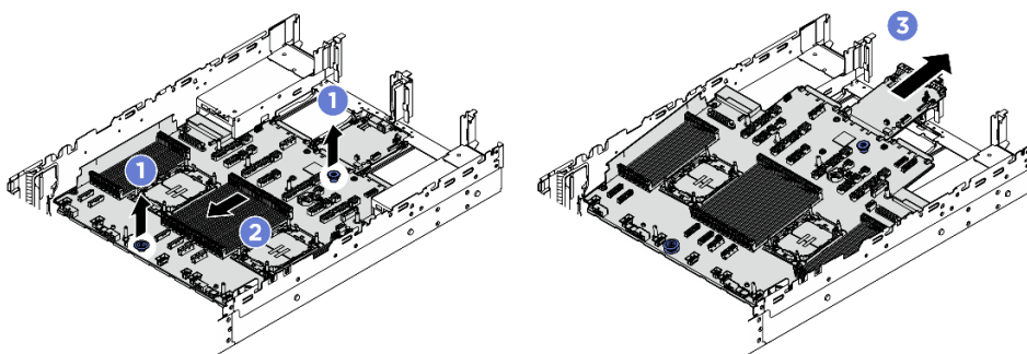
圖例 302. 卸下主機板組件
