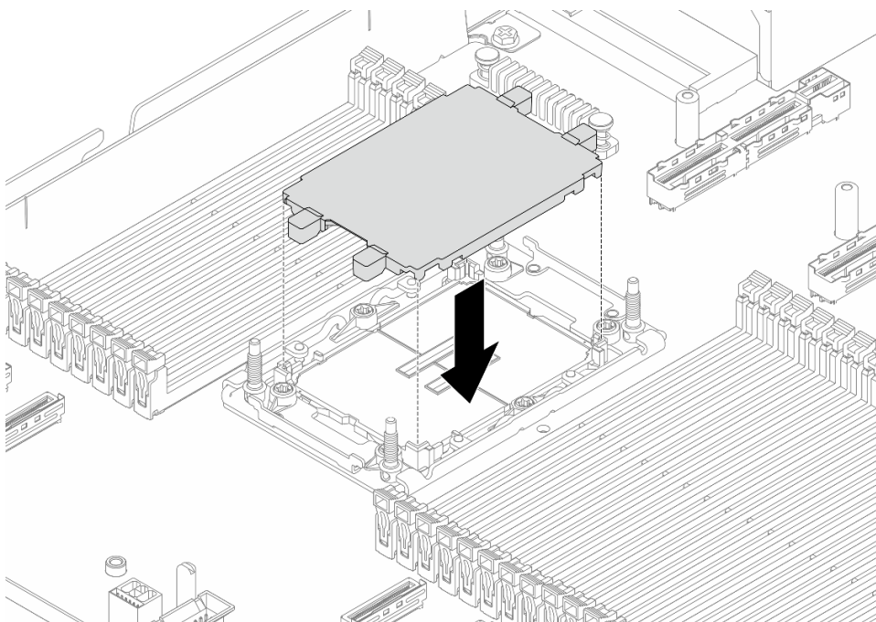
圖例 110. 安裝處理器插座蓋
