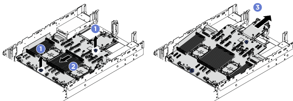
圖例 306. 卸下主機板組件
