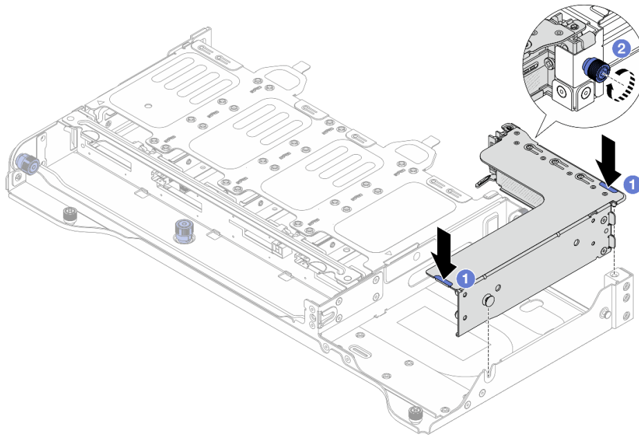
圖例 289. 安裝 2FH 擴充卡組件
