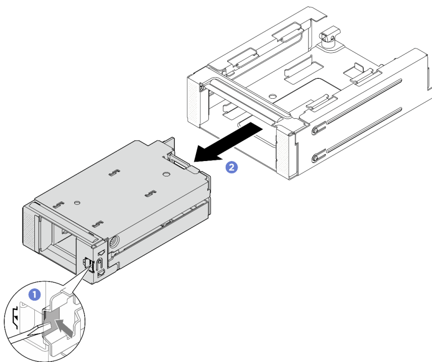
圖例 134. 從機架中卸下前方 M.2 框架
