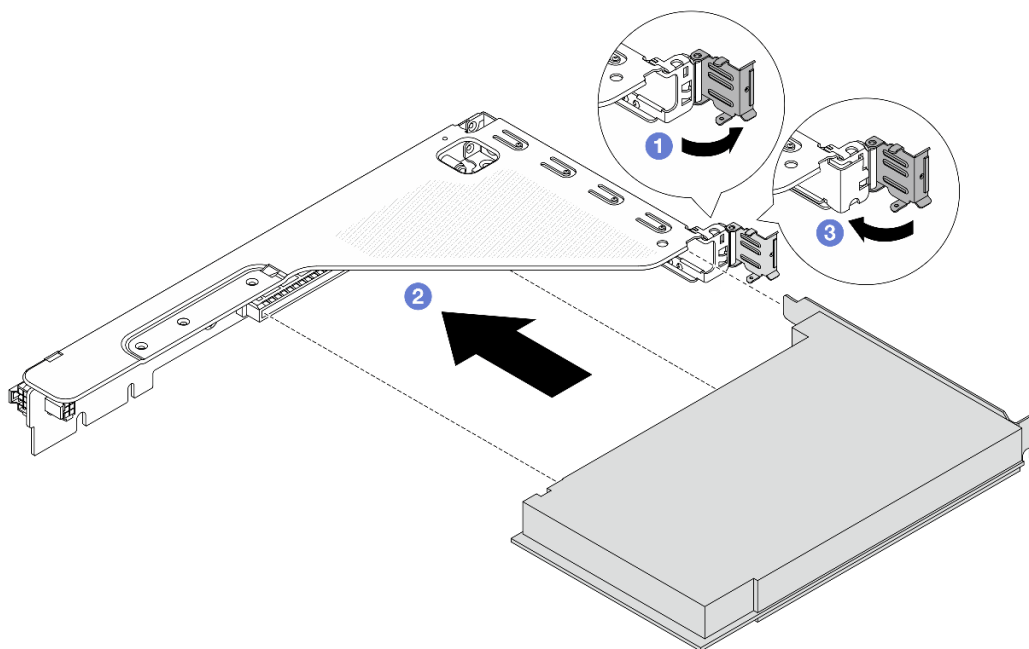
圖例 287. 在 1FH 擴充卡匣上安裝 PCIe 配接卡
