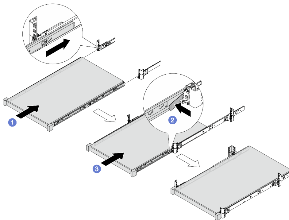
圖例 26. 安裝伺服器
