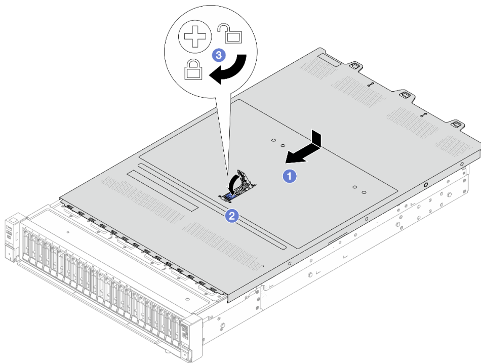
圖例 315. 安裝上蓋
