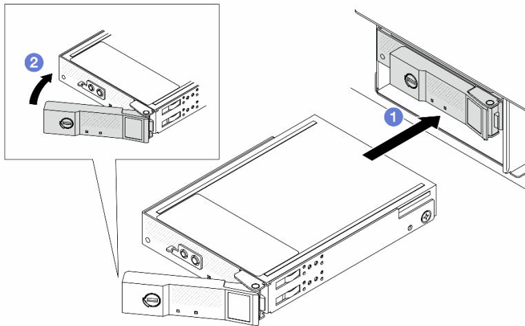
圖例 56. 安裝 E3.S CMM
