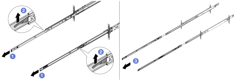
圖例 33. 拉出滑軌
