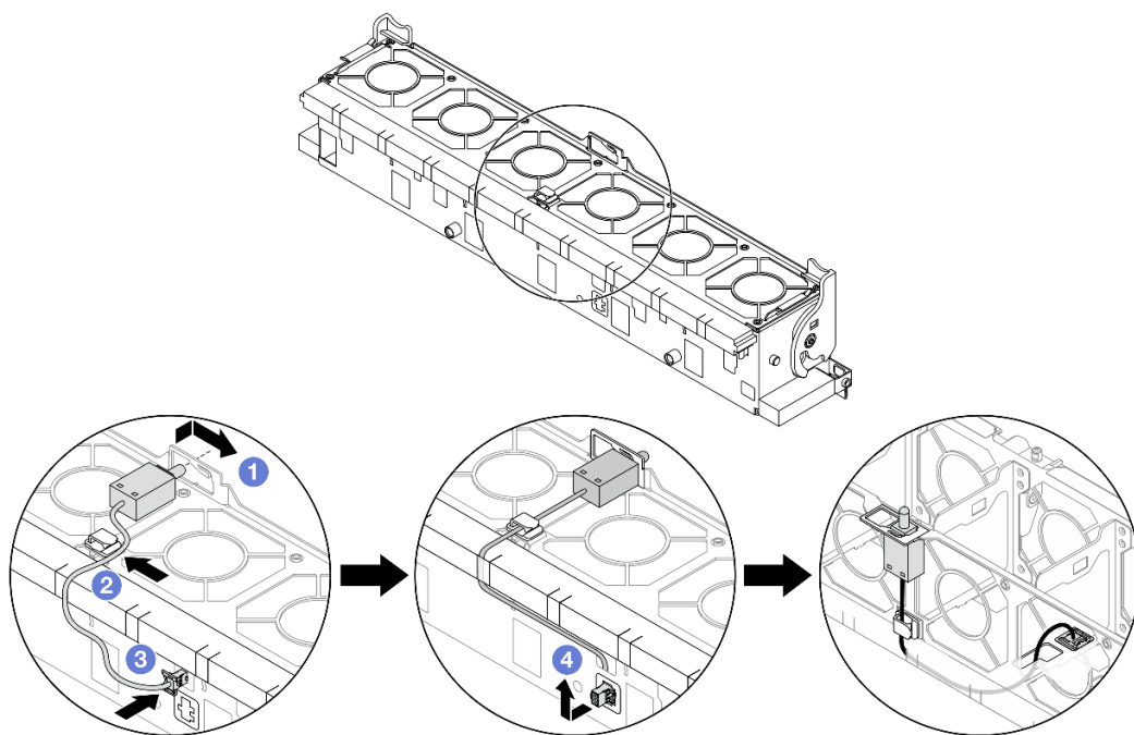
圖例 102. 安裝入侵開關
