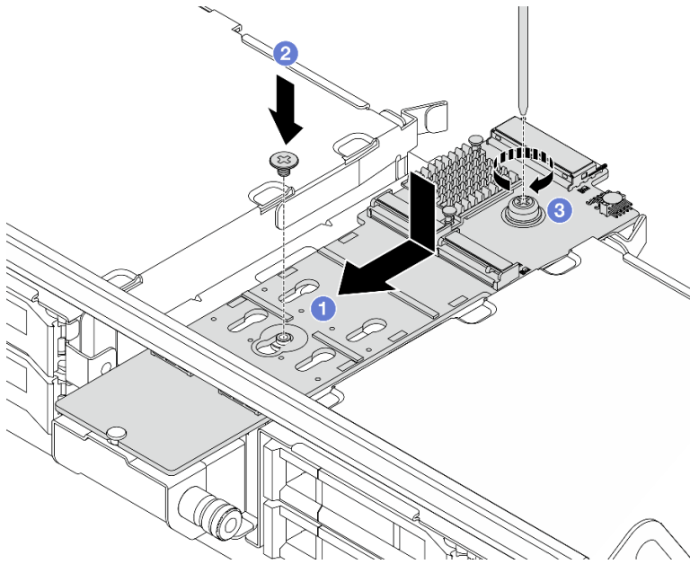
圖例 97. 將 M.2 背板安裝在中間框架上
