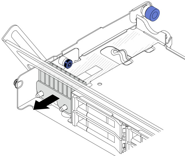
圖例 242. 卸下橡膠
