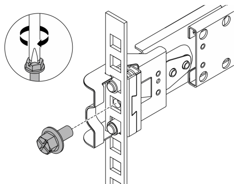
圖例 39. 將伺服器固定到機架背面
