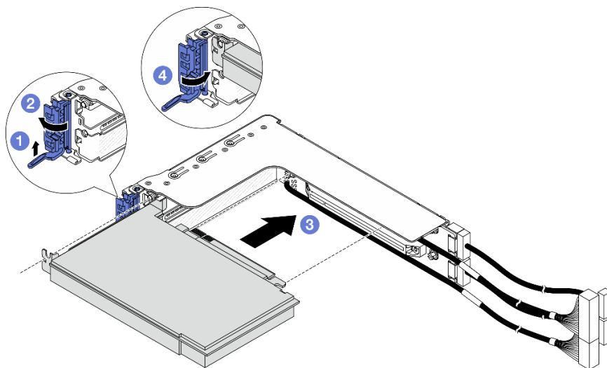
圖例 286. 在 2FH 擴充卡匣上安裝 PCIe 配接卡
