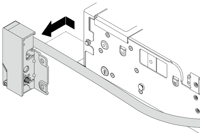
圖例 232. 卸下機架門鎖
