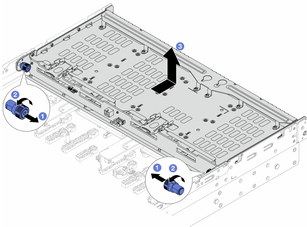
圖例 267. 卸下 4 x 3.5 吋背面框架
