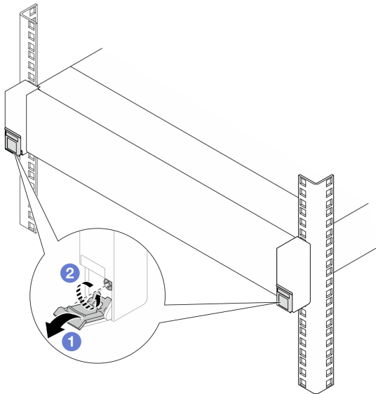
圖例 19. 鬆開機架門鎖上的螺絲
