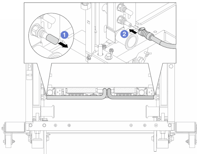
圖例 174. 安裝快速連接插件
