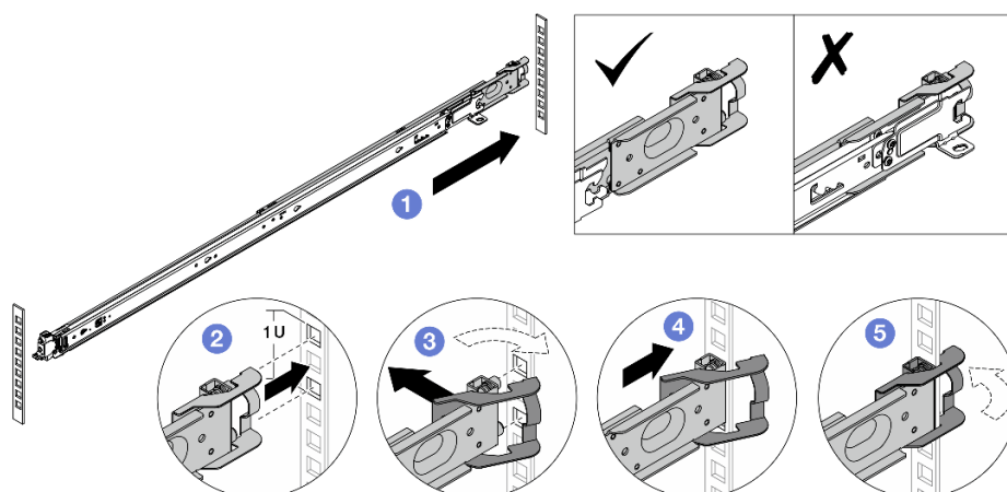
圖例 17. 安裝後方安裝插腳
