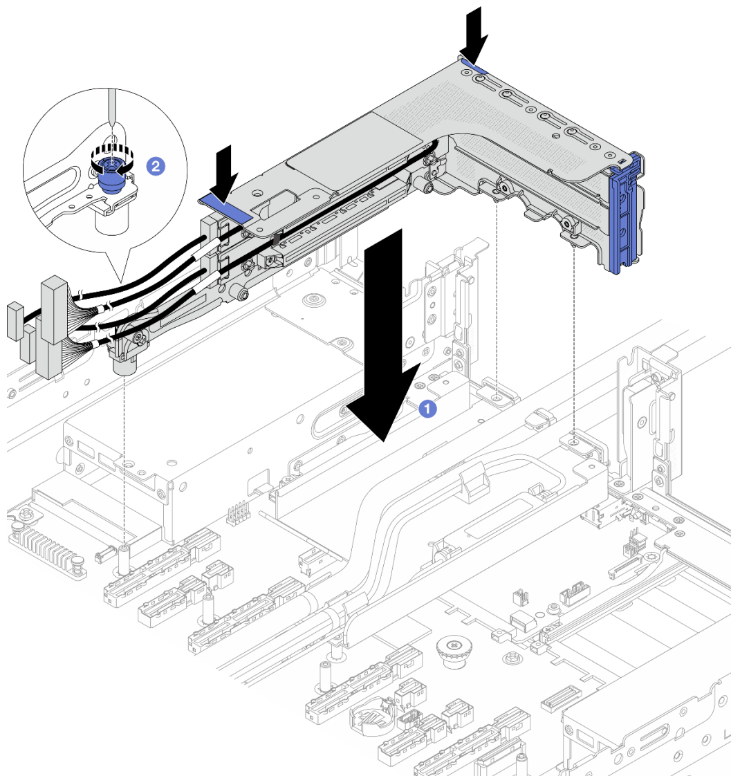
圖例 117. 安裝 3FH 擴充卡匣
