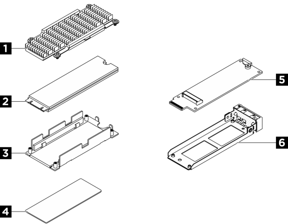
圖例 118. 熱抽換 M.2 硬碟組件的零件
