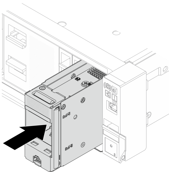
圖例 142. 將前方 M.2 框架安裝至機箱中
