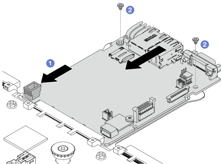
圖例 304. 將系統 I/O 板安裝在處理器板上
