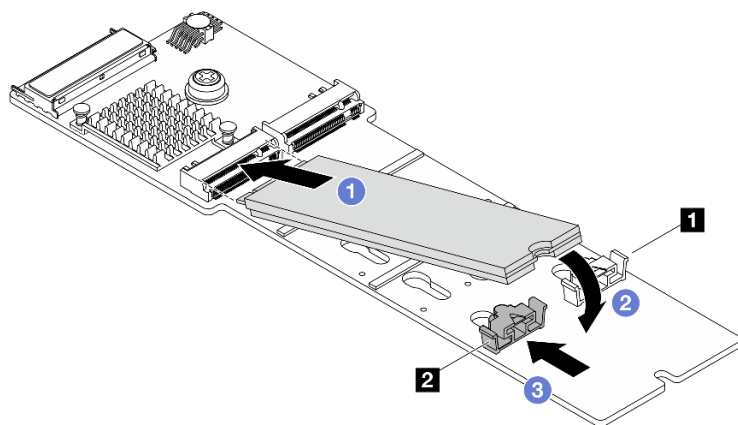
圖例 91. 安裝 M.2 硬碟
