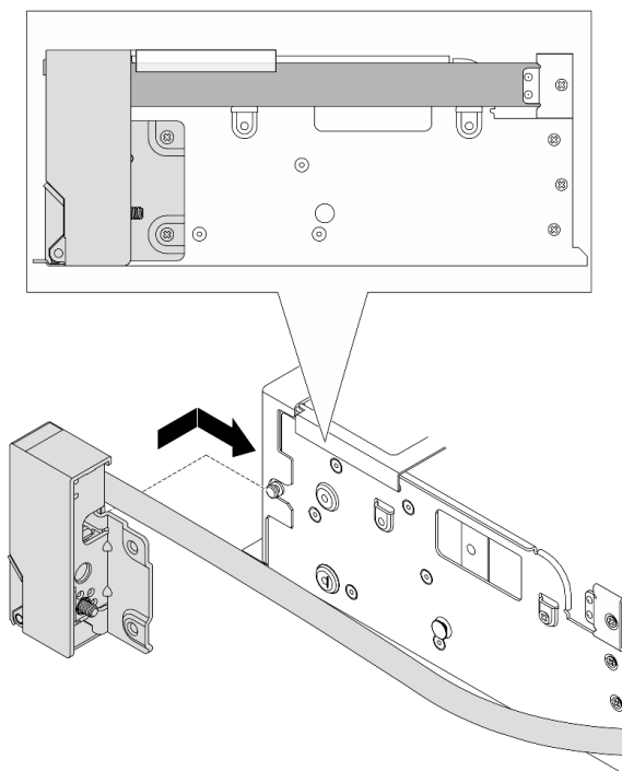
圖例 233. 安裝機架門鎖
