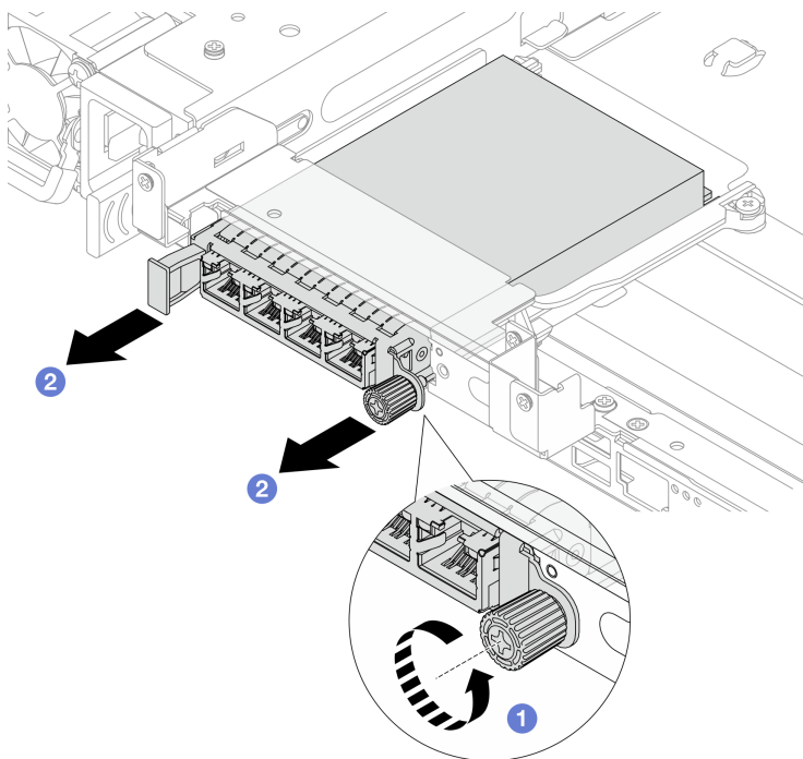
圖例 272. 卸下背面 OCP 模組
