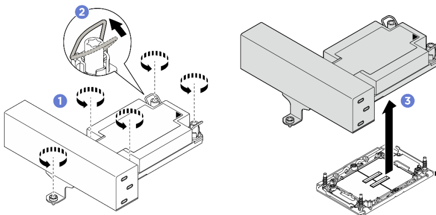
圖例 219. 卸下 1U T 形效能 PHM
