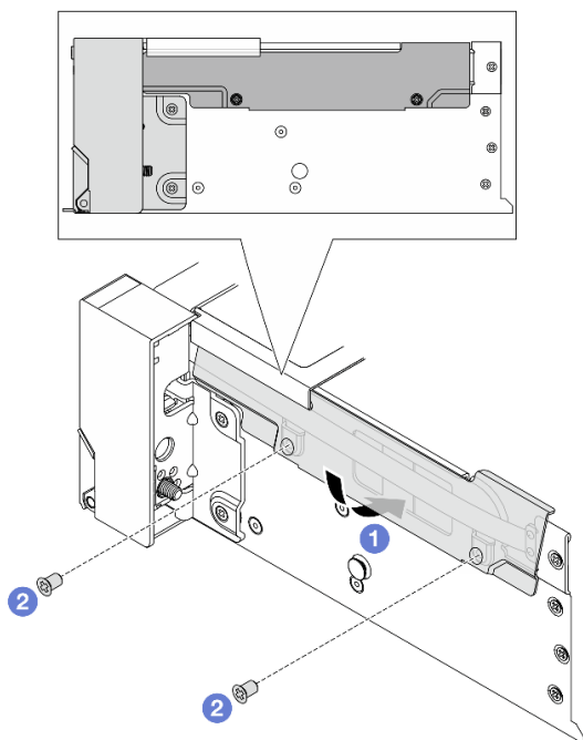
圖例 235. 安裝纜線固定夾
