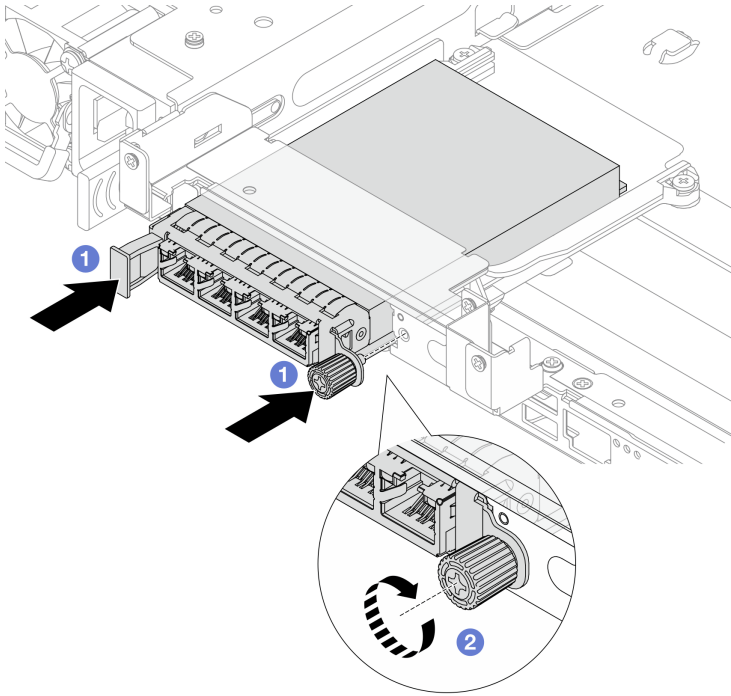
圖例 273. 安裝背面 OCP 模組
