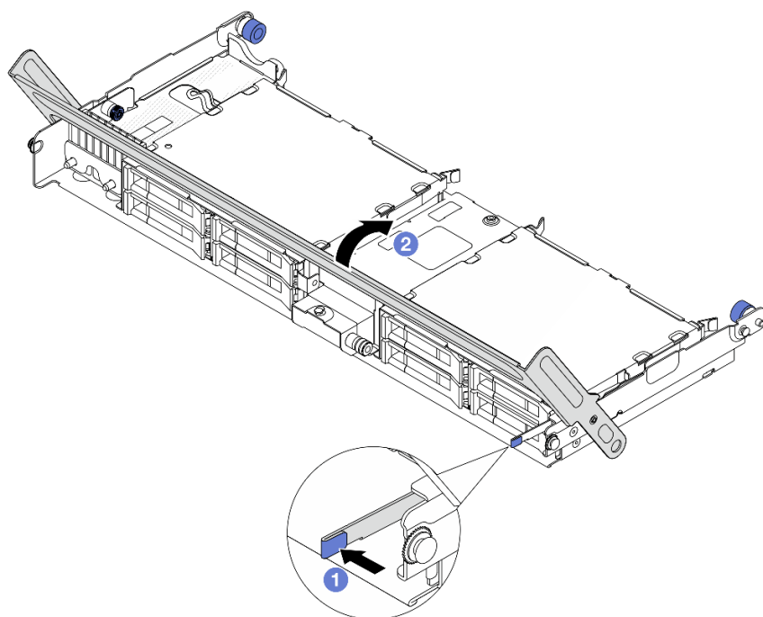
圖例 246. 關上框架把手
