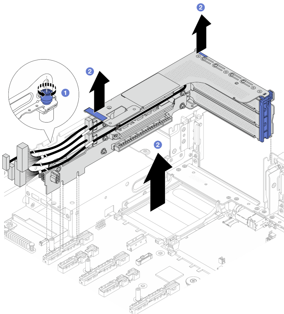
圖例 276. 卸下 3FH 擴充卡組件
