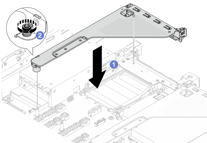
圖例 300. 安裝擴充卡組件
