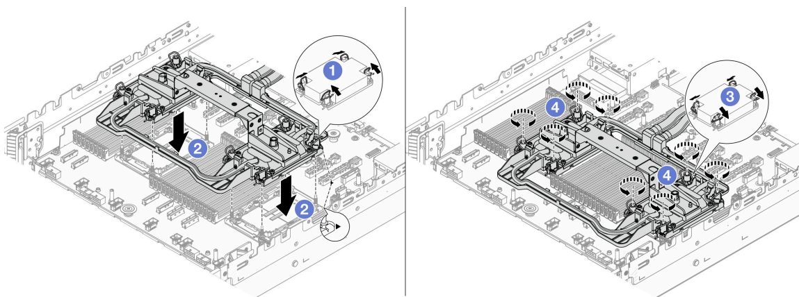
圖例 111. 安裝 Processor Neptune Core Module
