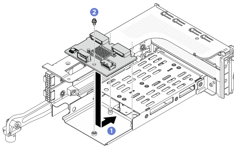
圖例 148. 將 M.2 背板安裝到 3FH M.2 擴充卡匣
