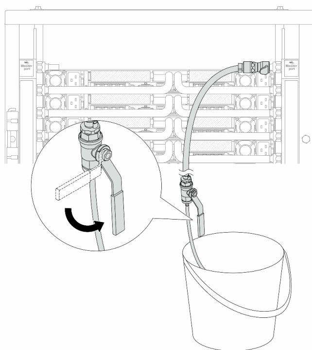
圖例 197. 開啟回流側的洩放閥門
