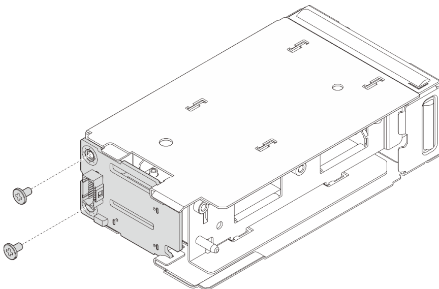
圖例 136. 卸下前方 M.2 開機背板
