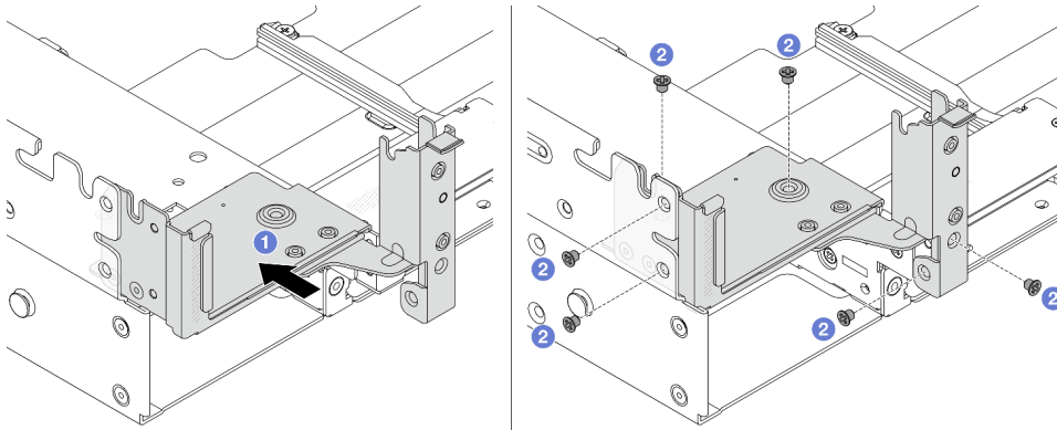
圖例 250. 安裝左側後壁托架
