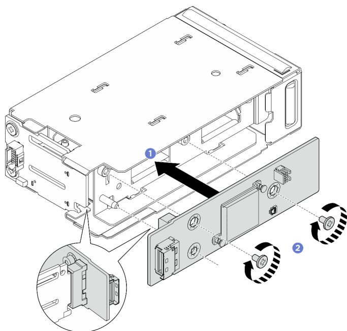
圖例 141. 安裝前方 M.2 控制器板
