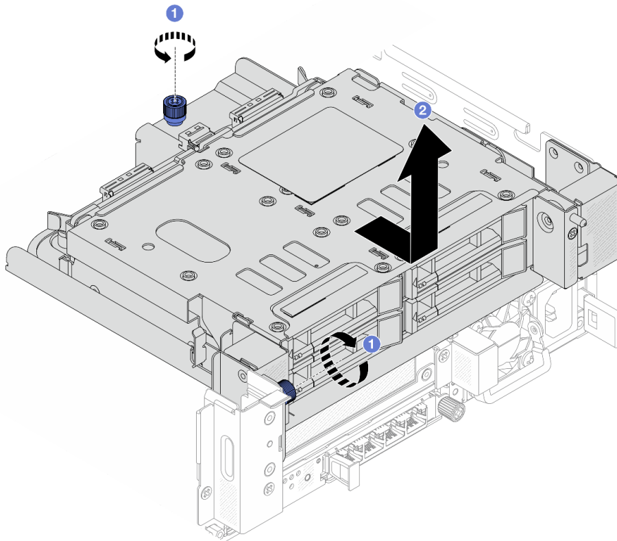
圖例 259. 卸下 4 x 2.5 吋背面框架
