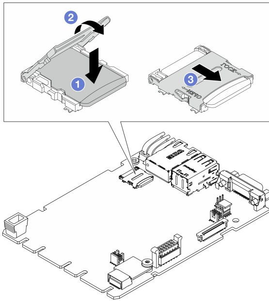
圖例 203. 安裝 MicroSD 卡
