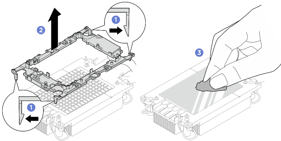
圖例 222. 將處理器支架與散熱槽分開
