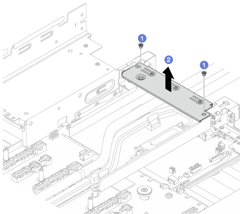
圖例 103. 卸下 1FH 托架
