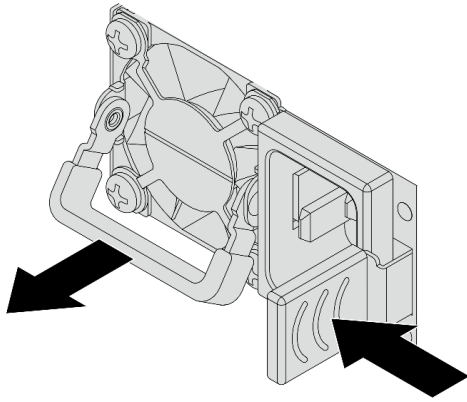
圖例 211. 卸下熱抽換電源供應器
