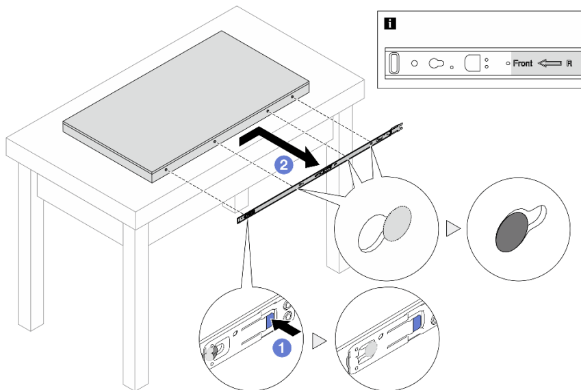
圖例 32. 卸下內滑軌
