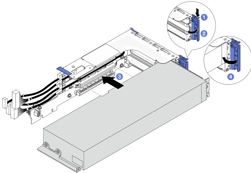
圖例 82. 安裝 GPU 配接卡
