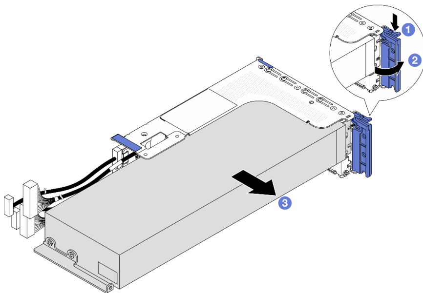
圖例 81. 卸下 GPU 配接卡
