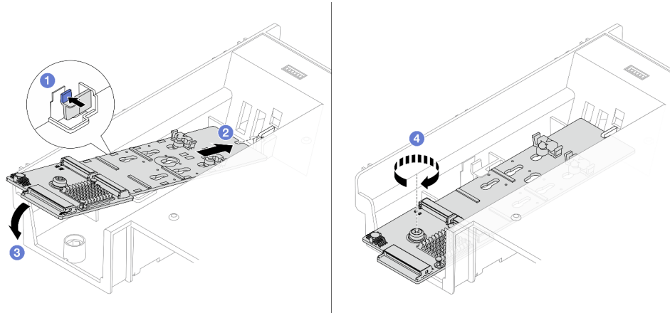
圖例 96. 將 M.2 背板安裝在空氣擋板上
