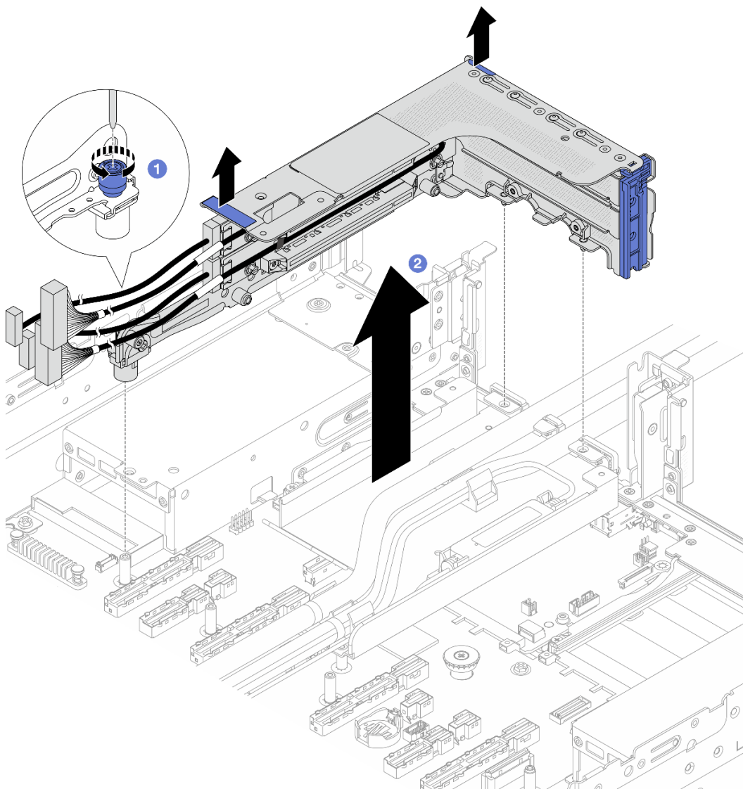
圖例 104. 卸下 3FH 擴充卡匣
