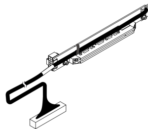
圖例 11. 含電源接頭的含纜線擴充卡 ( Gen5 x16 , 300 公釐 , 插槽 4/7 )
