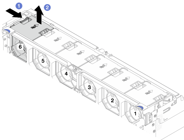
圖例 310. 卸下系統風扇
