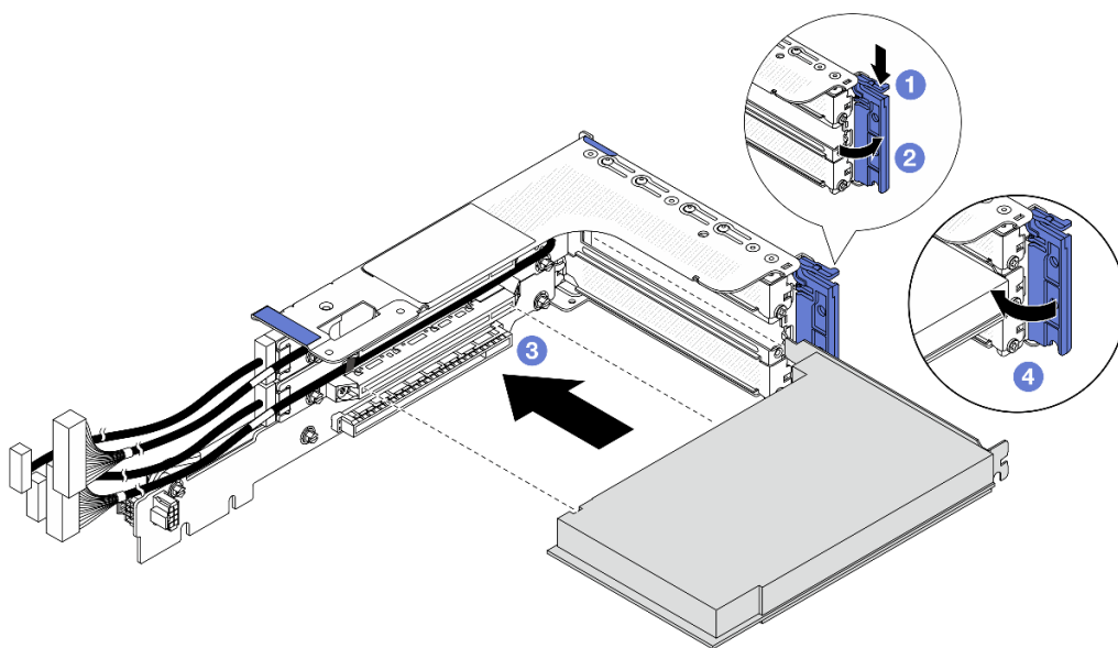
圖例 285. 在 3FH 擴充卡匣上安裝 PCIe 配接卡
