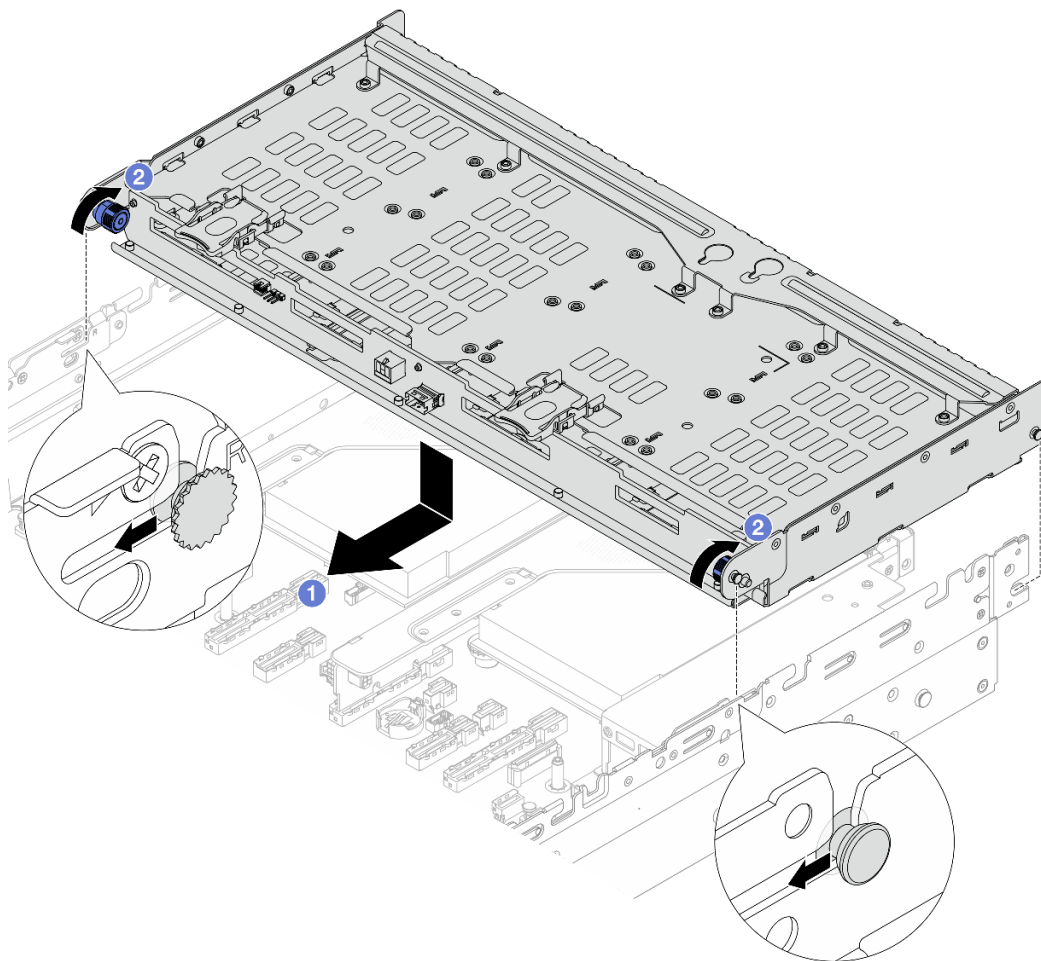
圖例 270. 安裝 4 x 3.5 吋背面框架
