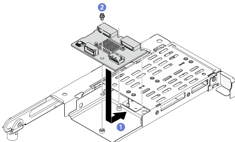
圖例 149. 將 M.2 背板安裝到 1FH M.2 擴充卡匣
