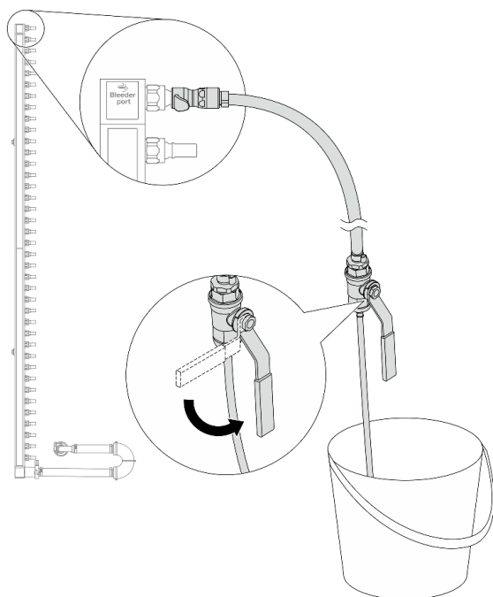
圖例 163. 開啟洩放閥門
