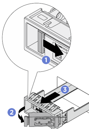
圖例 121. 卸下 M.2 硬碟匣
