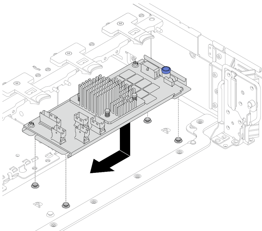
圖例 87. 安裝內部 CFF 配接卡
