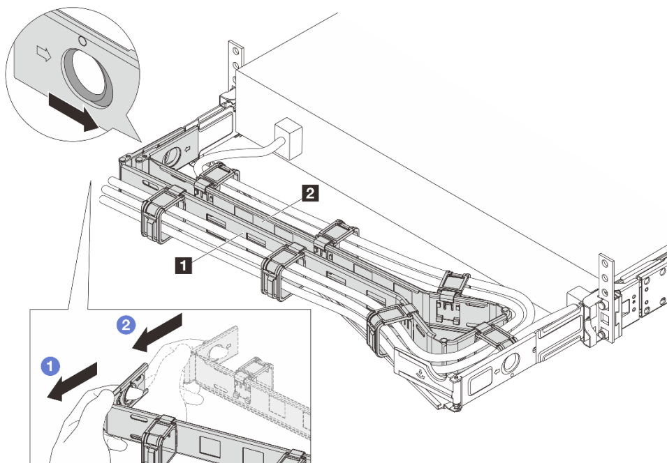
圖例 210. 卸下左側
