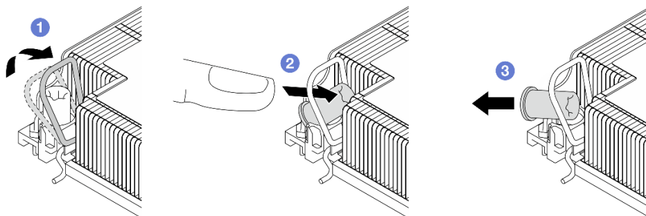
圖例 84. 從散熱槽卸下 Torx T30 螺帽
