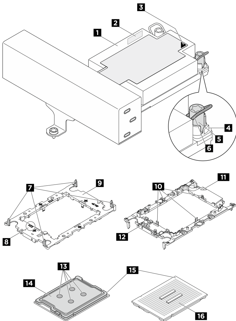
圖例 223. PHM 元件
