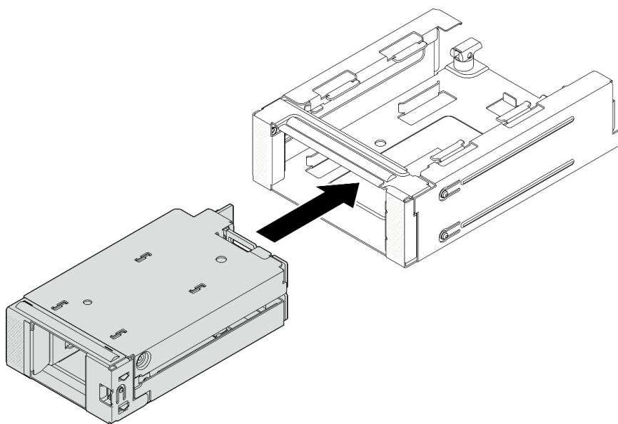
圖例 143. 將前方 M.2 框架安裝至機架中
