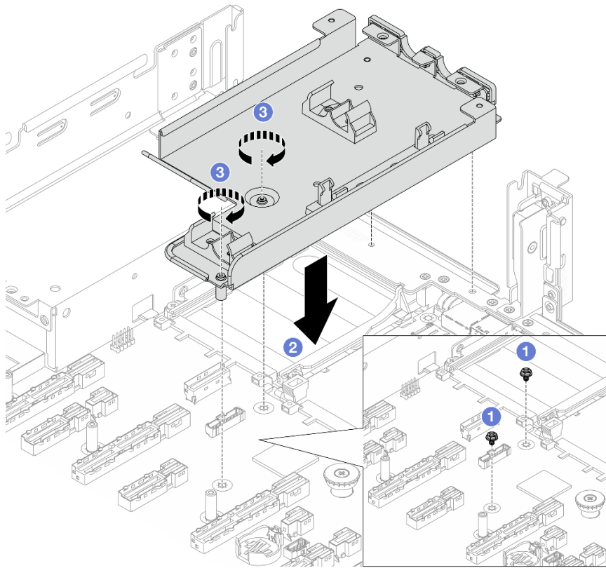
圖例 108. 安裝水管固定器
