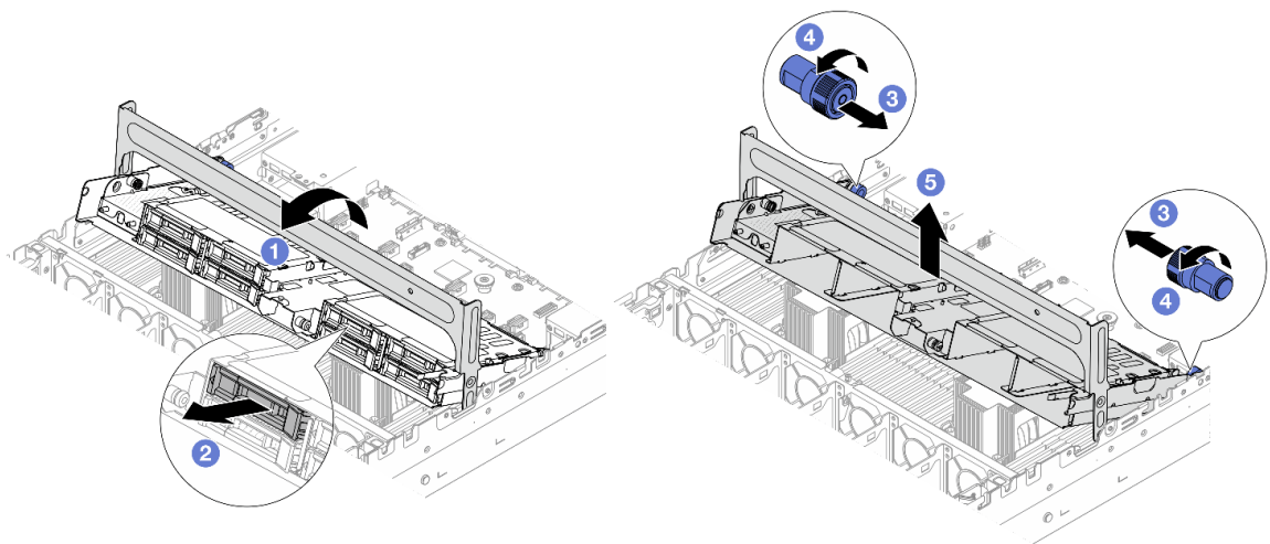
圖例 204. 卸下中間框架
