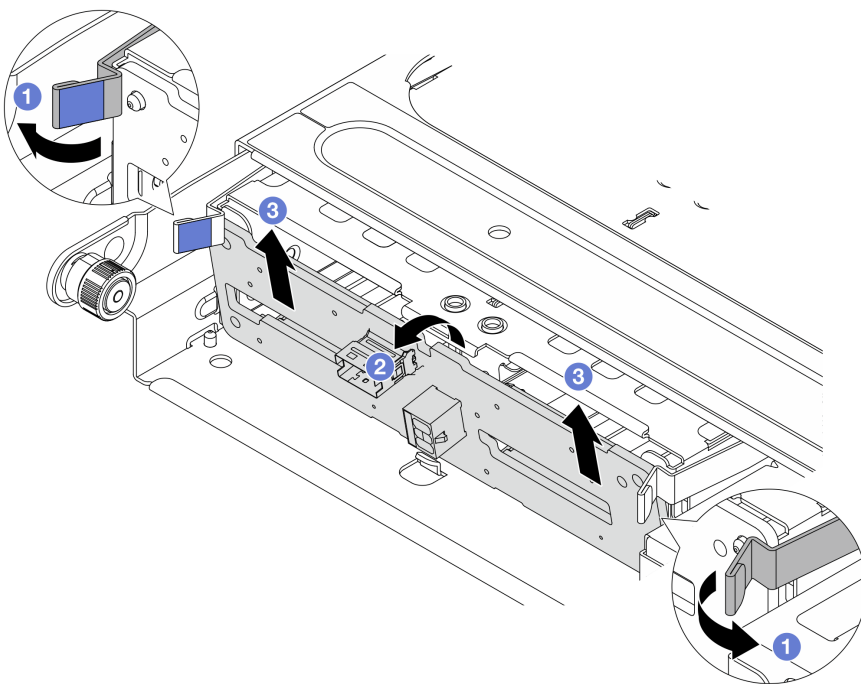
圖例 205. 卸下 2.5 吋中間硬碟背板
