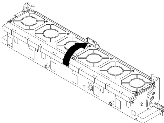
圖例 100. 旋轉風扇機盒
