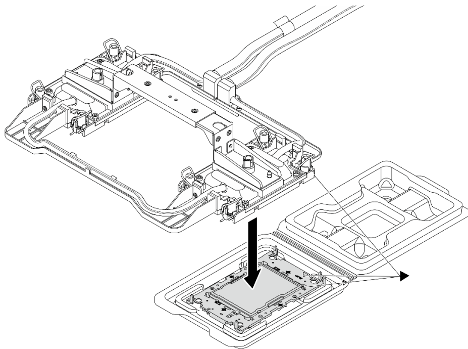
圖例 109. 安裝處理器
