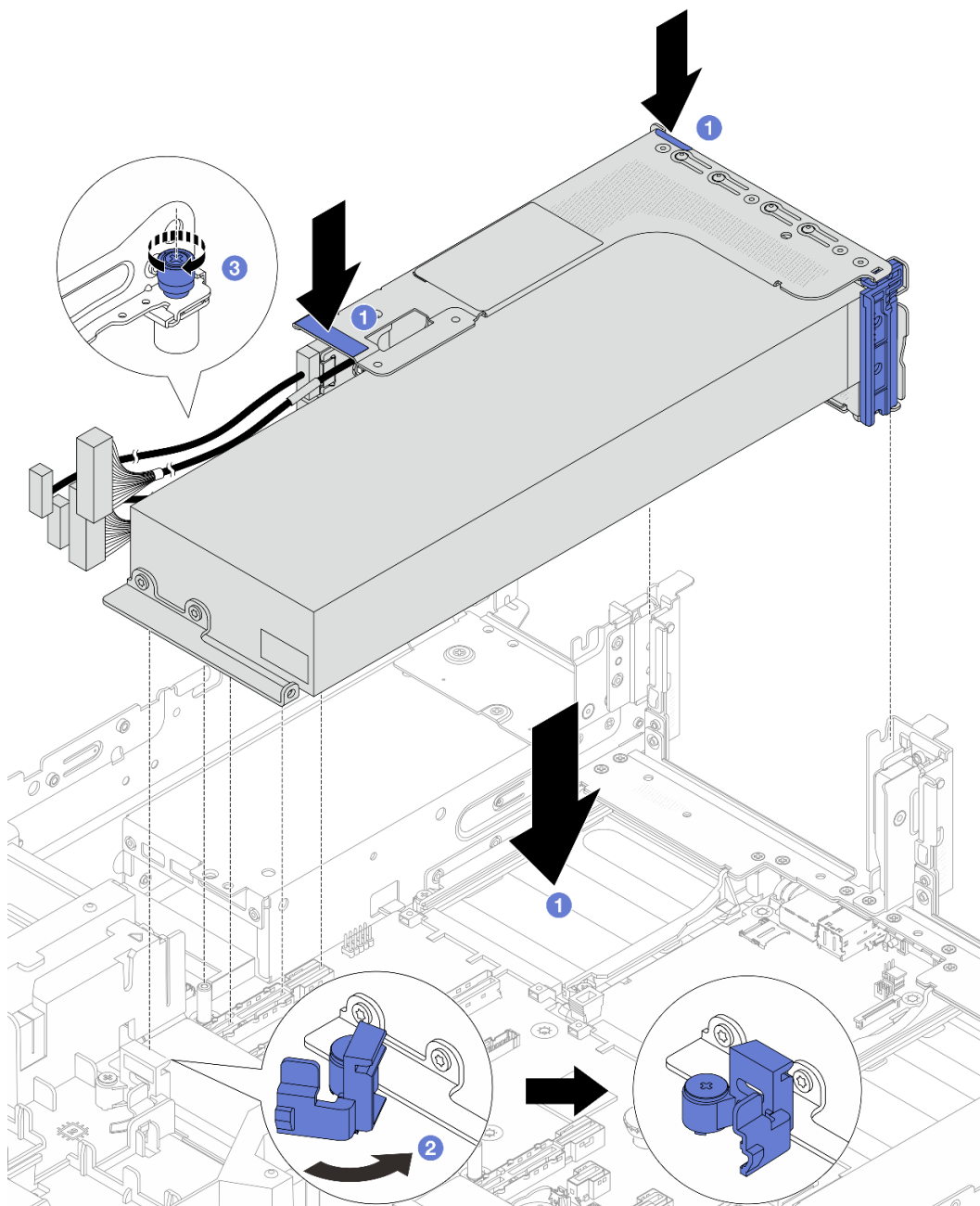
圖例 83. 安裝配備 GPU 配接卡的擴充卡組件
