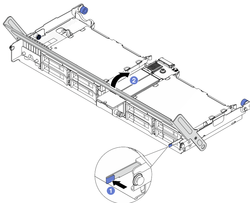
圖例 98. 關上中間框架的把手
