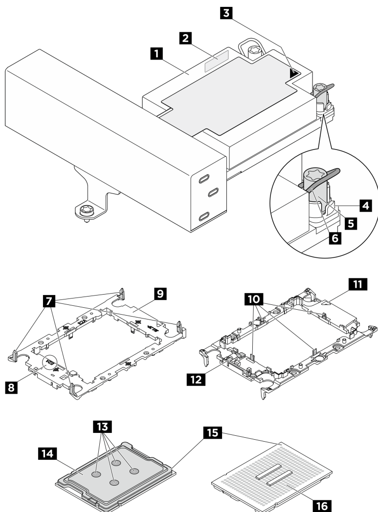
圖例 217. PHM 元件
