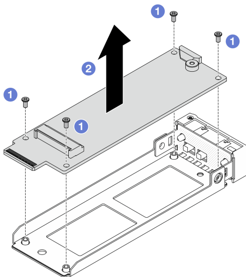
圖例 124. 移除 M.2 轉插卡
