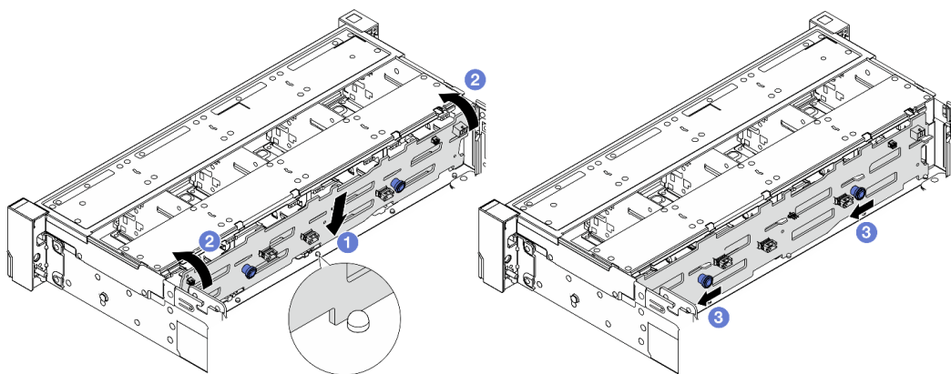
圖例 79. 安裝前方 3.5 吋硬碟背板
