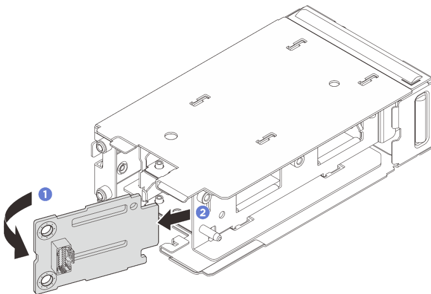
圖例 137. 卸下前方 M.2 開機背板
