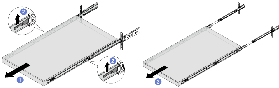
圖例 31. 拉出伺服器
