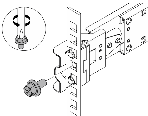
圖例 12. 卸下 M6 螺絲
