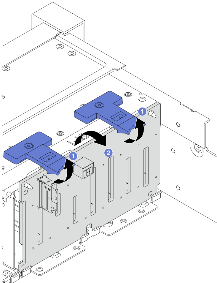
圖例 76. 卸下前方 2.5 吋硬碟背板
