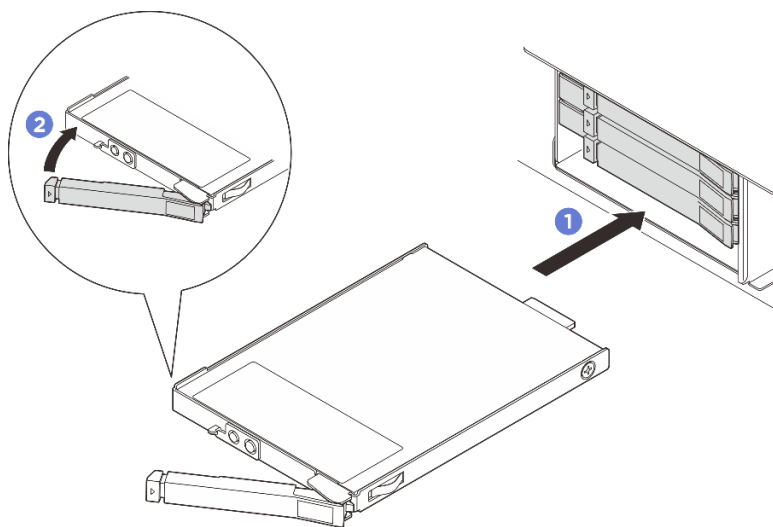
圖例 68. 安裝 E3.S 熱抽換硬碟
