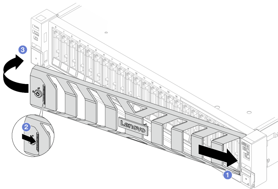
圖例 293. 安裝安全擋板
