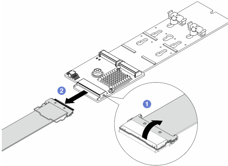
圖例 92. 拔掉 M.2 纜線
