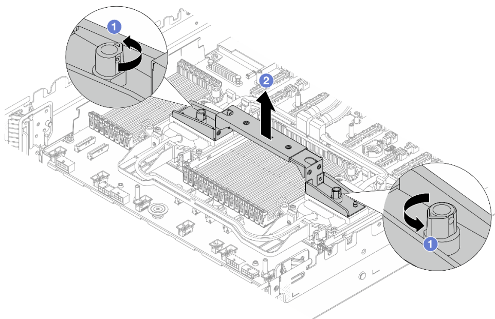
圖例 112. 卸下模組把手
