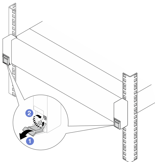
圖例 38. 將伺服器固定到機架正面
