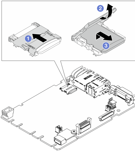
圖例 202. 卸下 MicroSD 卡
