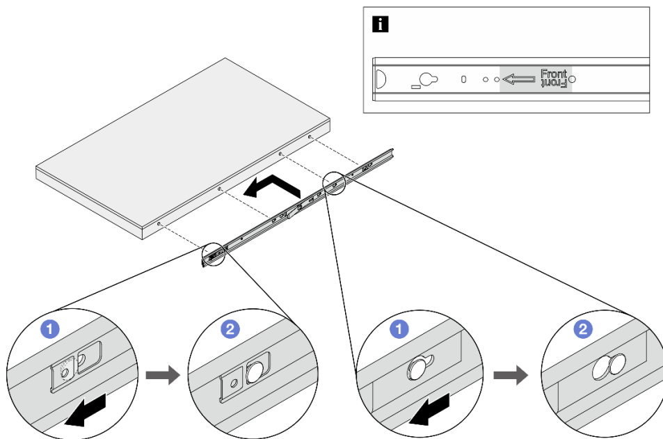
圖例 24. 安裝內滑軌
