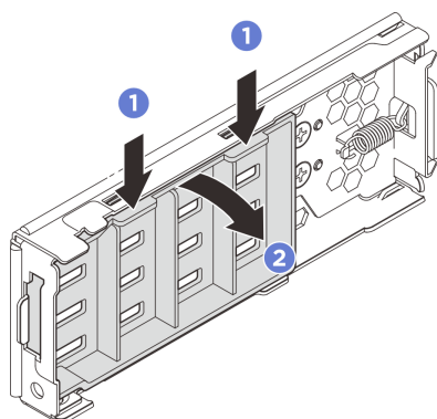
圖例 58. 卸下內板
