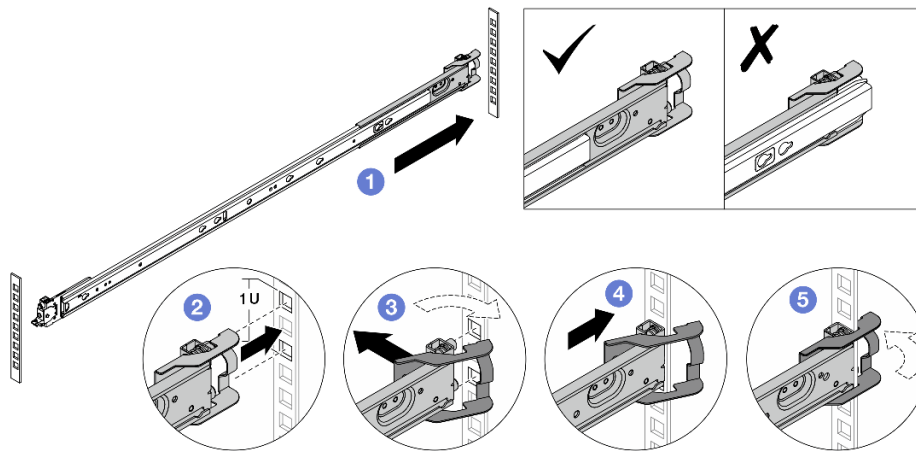
圖例 15. 安裝後方安裝插腳
