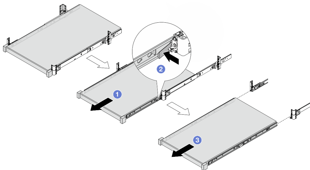
圖例 21. 卸下伺服器
