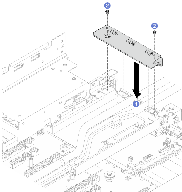
圖例 116. 安裝 1FH 托架
