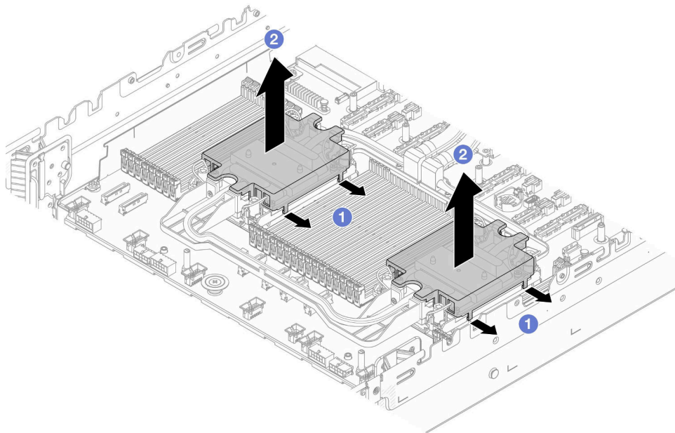
圖例 334. 拆下水冷板蓋
