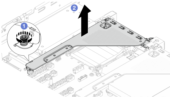
圖例 295. 卸下擴充卡組件
