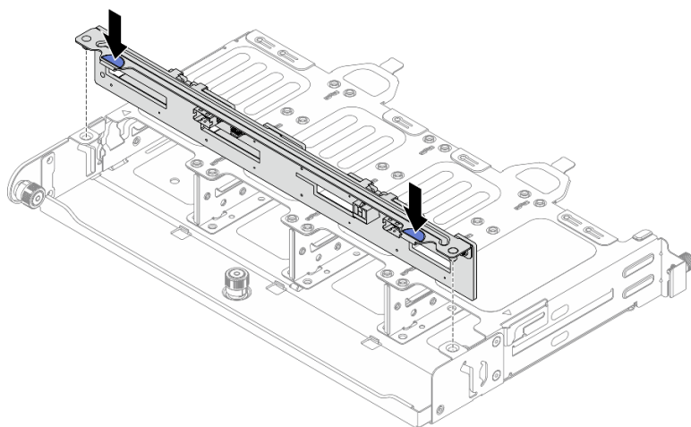
圖例 265. 安裝 8 x 2.5 吋後方硬碟背板
