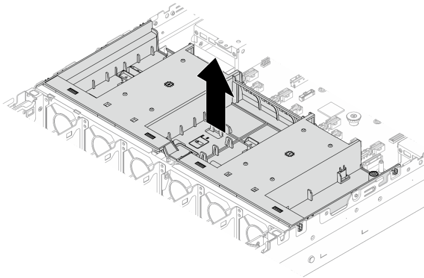
圖例 42. 卸下空氣擋板
