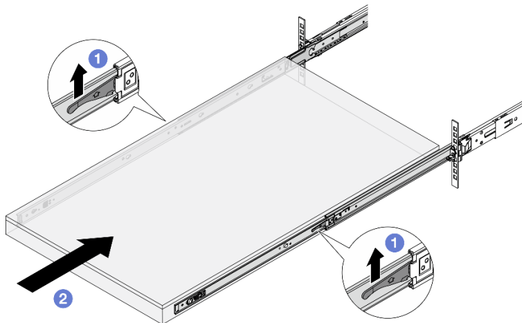
圖例 37. 鎖定滑軌，並將伺服器滑入
