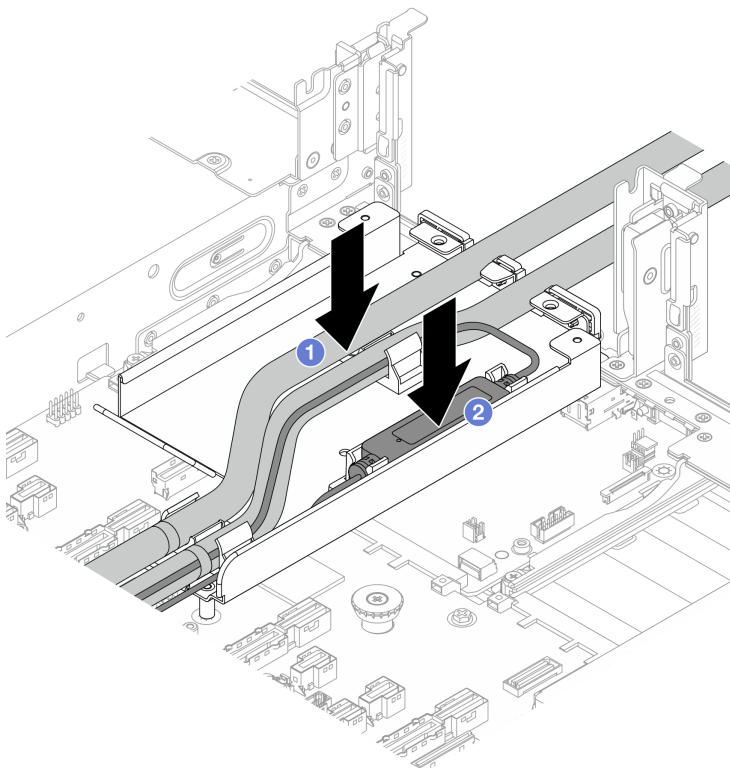
圖例 114. 放置水管和洩漏偵測感應器模組
