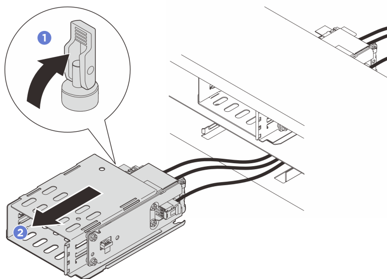
圖例 72. 卸下 E3.S 1T 框架
