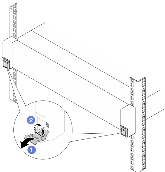
圖例 29. 使伺服器脫離機架
