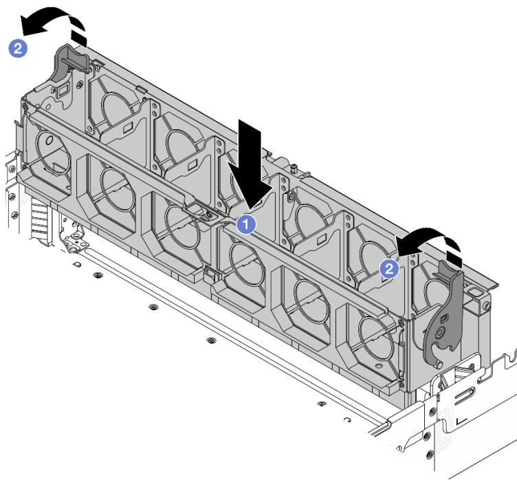
圖例 313. 安裝系統風扇機盒
