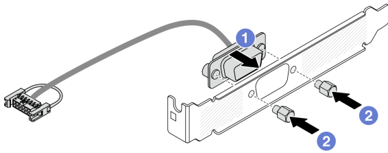
圖例 298. 組裝序列埠模組
