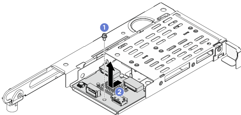
圖例 147. 從 1FH M.2 擴充卡匣中卸下 M.2 背板
