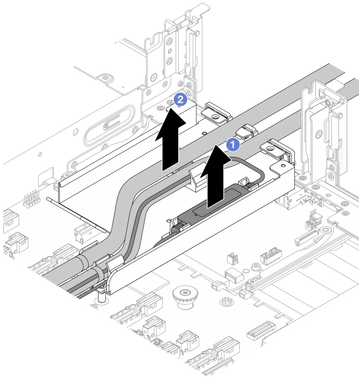
圖例 105. 卸下軟管和洩漏偵測感應器模組
