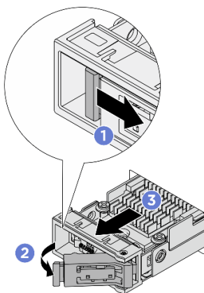
圖例 119. 卸下熱抽換 M.2 硬碟組件
