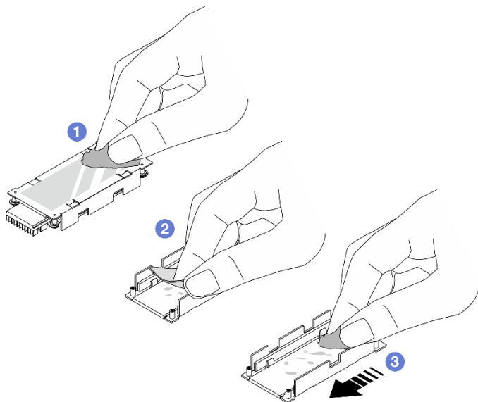
圖例 126. 清潔散熱槽和底板
