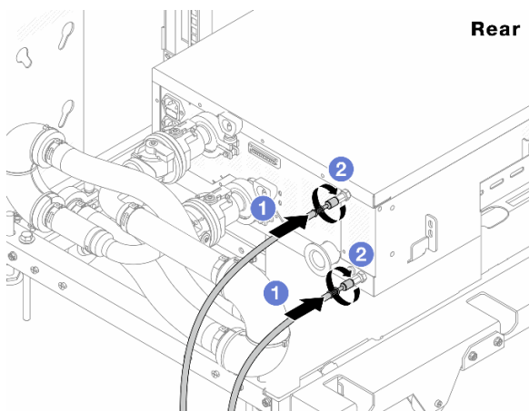
圖例 173. CDU 的背面
