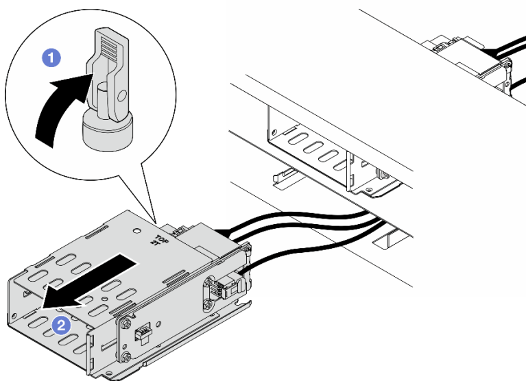
圖例 60. 卸下 E3.S 2T 框架
