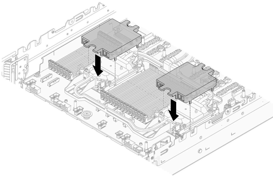
圖例 113. 安裝水冷板蓋
