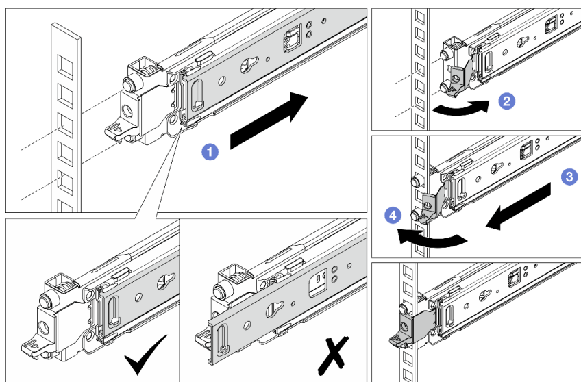
圖例 18. 安裝前方安裝插腳
