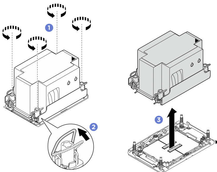
圖例 218. 卸下 2U 標準 PHM
