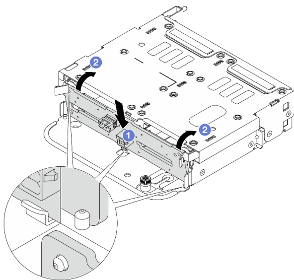
圖例 256. 安裝 4 x 2.5 吋後方硬碟背板
