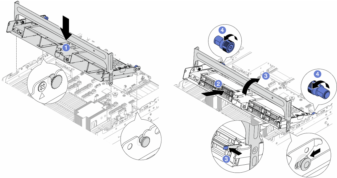
圖例 208. 安裝中間框架和硬碟
