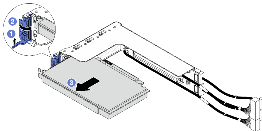
圖例 280. 從 2FH 擴充卡匣卸下 PCIe 配接卡
