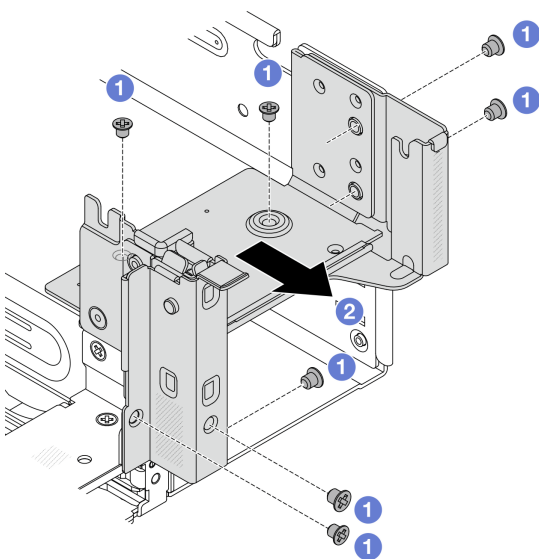
圖例 249. 卸下右側後壁托架
