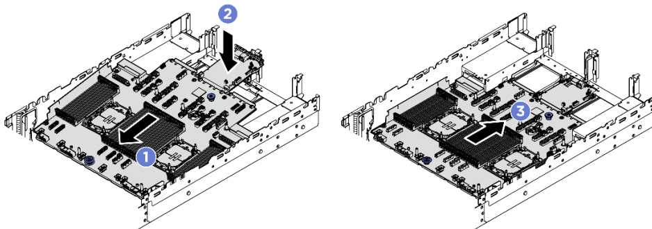
圖例 309. 安裝主機板組件
