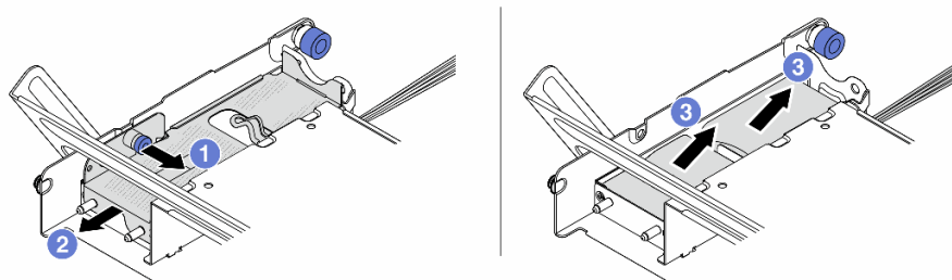
圖例 243. 從中間框架卸下 RAID 快閃記憶體電源模組
