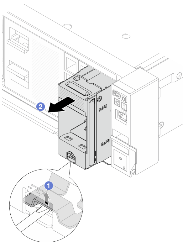
圖例 133. 從機箱中卸下前方 M.2 框架
