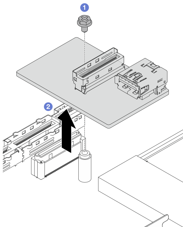
圖例 316. 卸下 USB I/O 板
