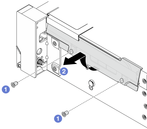
圖例 230. 卸下纜線固定夾
