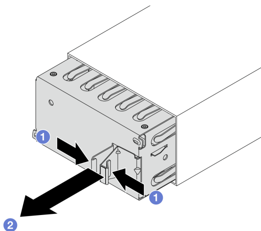
圖例 214. 卸下電源供應器填充板
