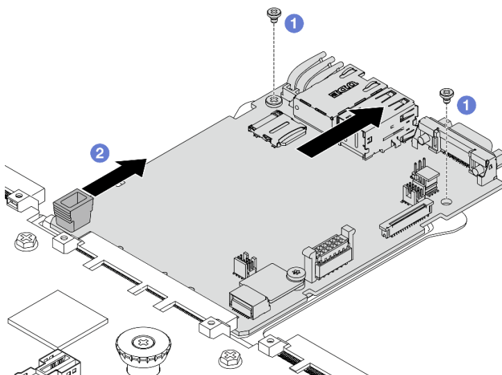
圖例 307. 將系統 I/O 板與處理器板分開
