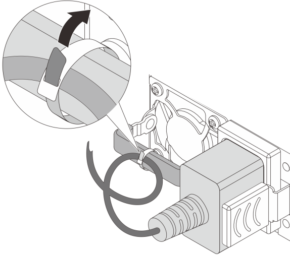
圖例 216. 佈線和固定電源線
