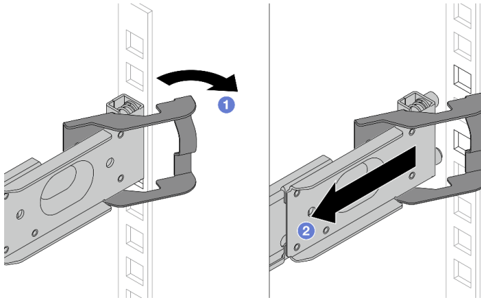
圖例 14. 從後方卸下滑軌
