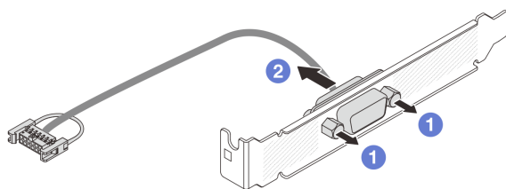
圖例 297. 拆卸序列埠模組
