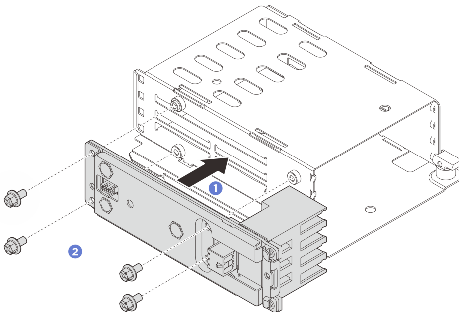
圖例 74. 安裝背板組件
