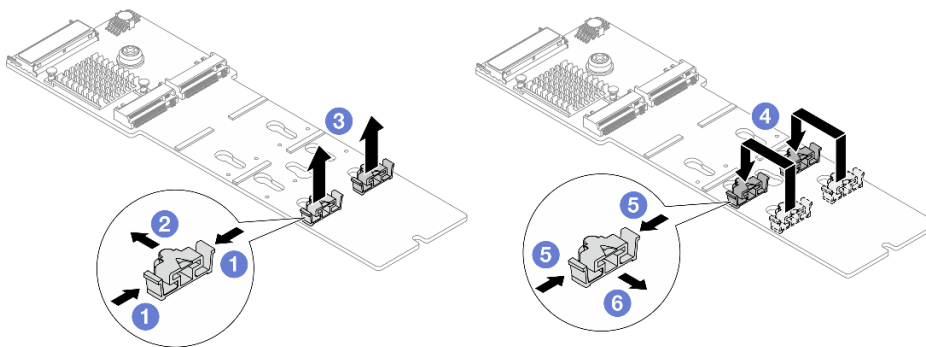
圖例 89. 調整 M.2 固定器
