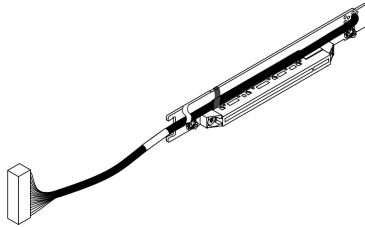
圖例 8. 含纜線擴充卡 ( Gen5 x8 , 350 公釐 )
