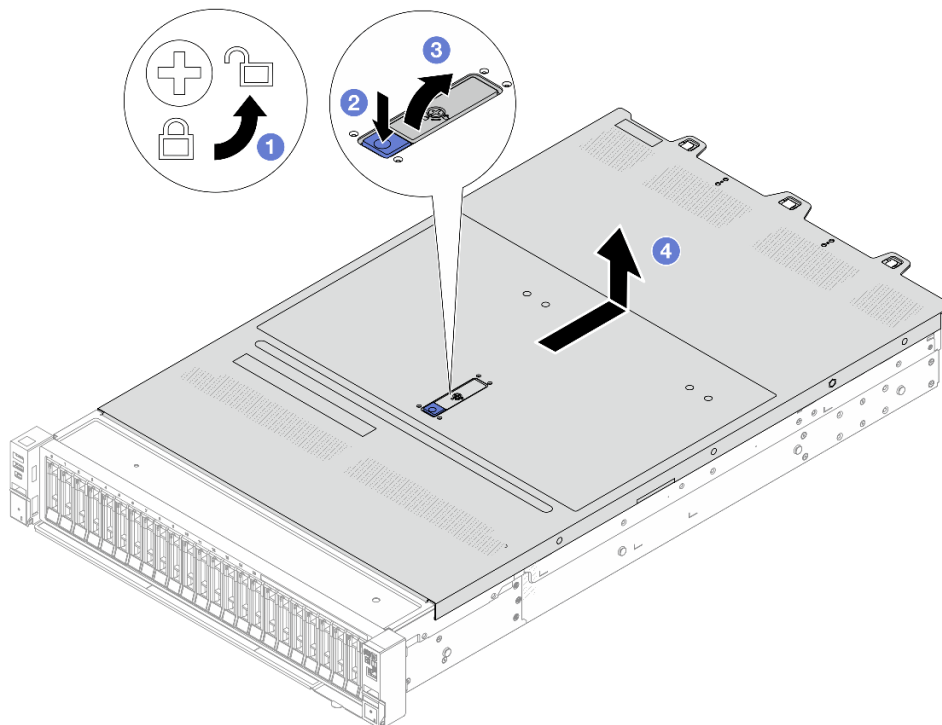
圖例 314. 卸下上蓋
