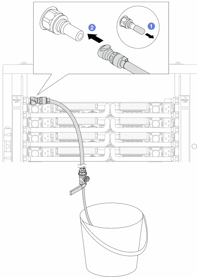
Abbildung 174. Installieren des Ablasssatzes an der Zulaufseite
