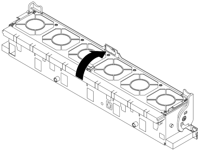
Abbildung 86. Drehen des Lüfterrahmens
