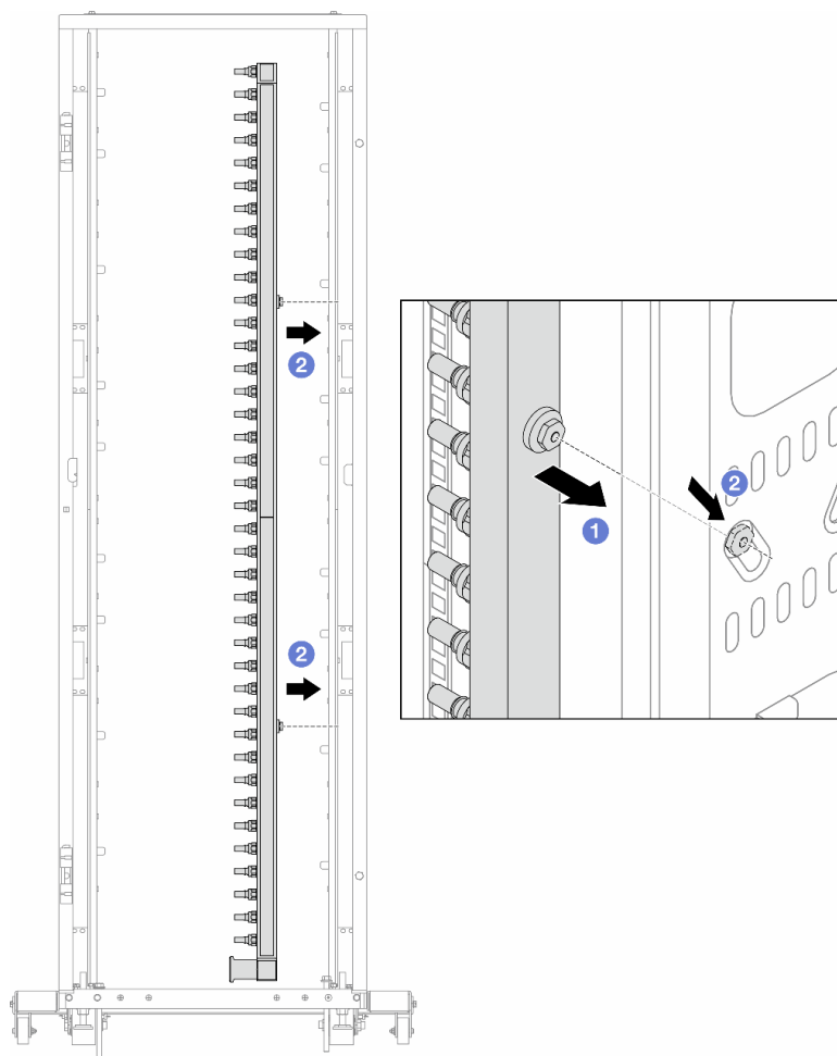
Abbildung 149. Installieren der Leitung
