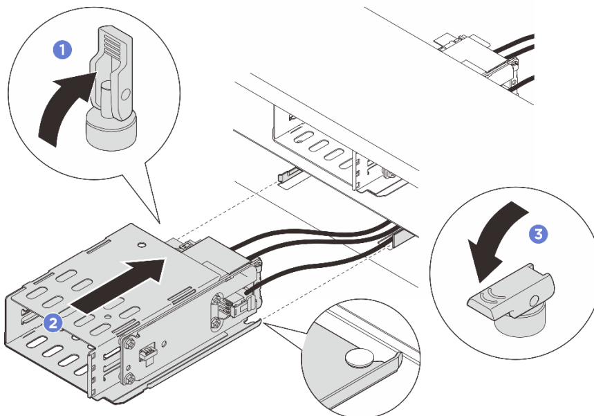
Abbildung 51. Installieren der E3.S-1T-Halterung
