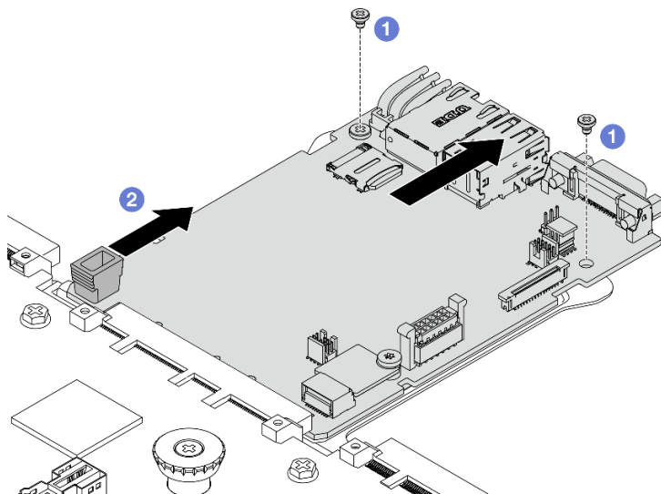
Abbildung 236. Trennen der System-E/A-Platine von der Prozessorplatine
