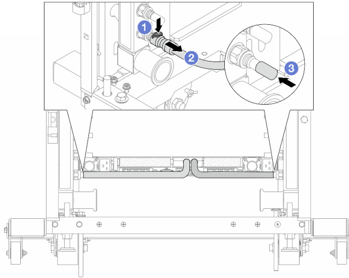
Abbildung 164. Entfernen der Schnellanschlüsse
