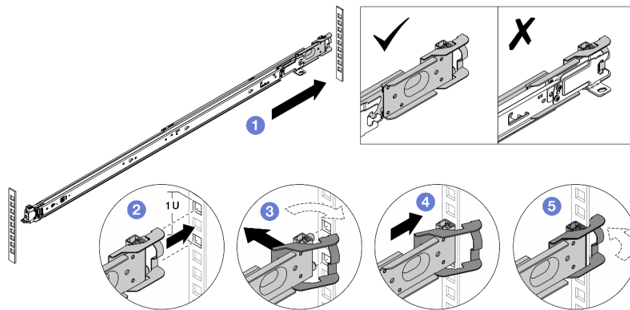
Abbildung 5. Installieren der hinteren Befestigungsstifte
