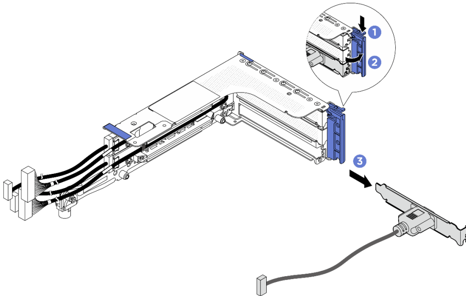
Abbildung 225. Entfernen des seriellen Anschlussmoduls
