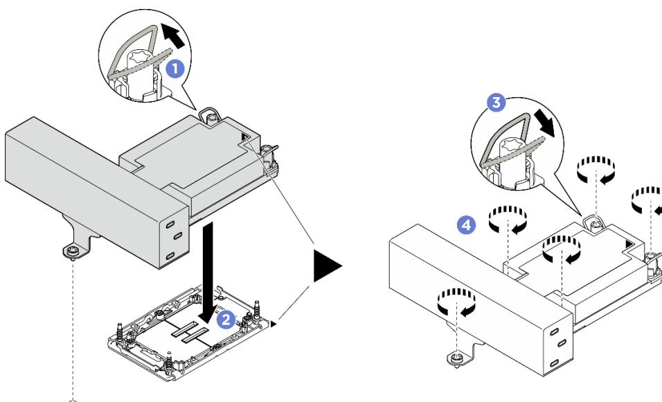
Abbildung 198. Installieren eines T-förmigen 1U-Hochleistungs-PHMs
