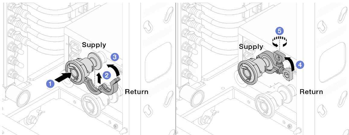
Abbildung 151. Installieren der Kugelhähne
