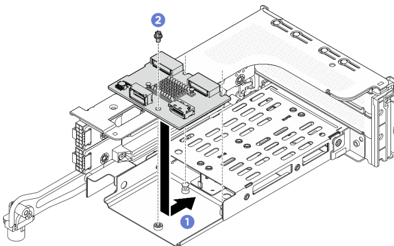
Abbildung 131. Installieren der M.2-Rückwandplatine in einem 3FH-M.2-Adapterrahmen
