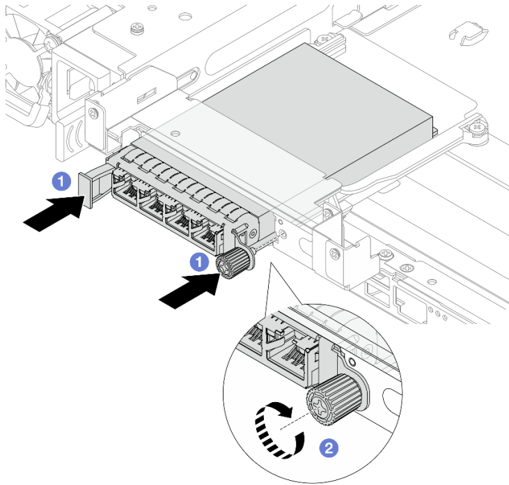
Abbildung 209. Installieren des hinteren OCP-Moduls
