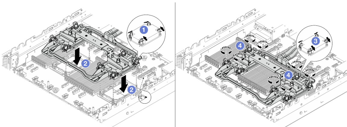
Abbildung 97. Installieren der Processor Neptune Core Module
