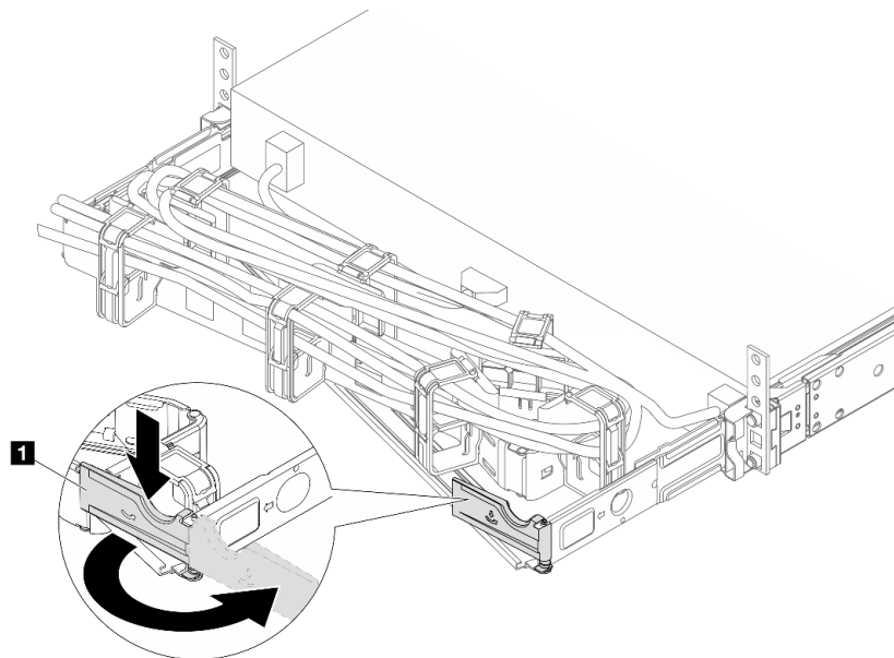
Abbildung 67. Einstellen der rechten Seite
