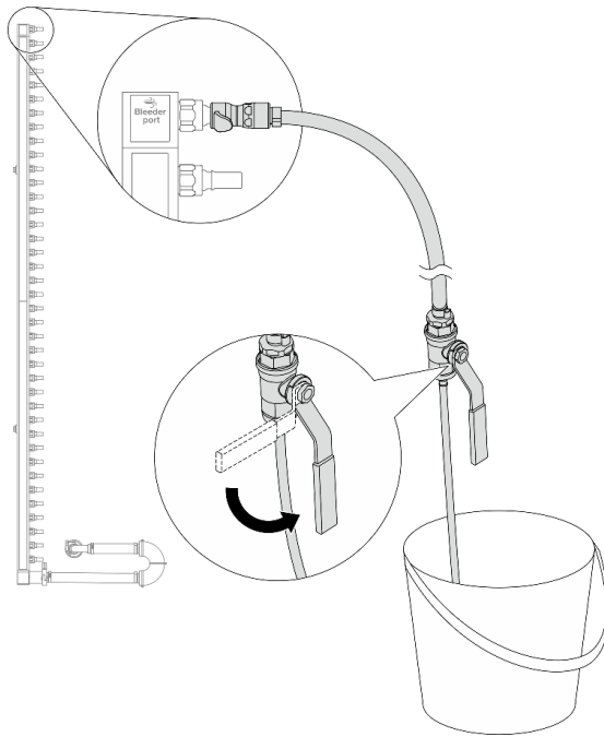
Abbildung 145. Öffnen des Ablassventils
