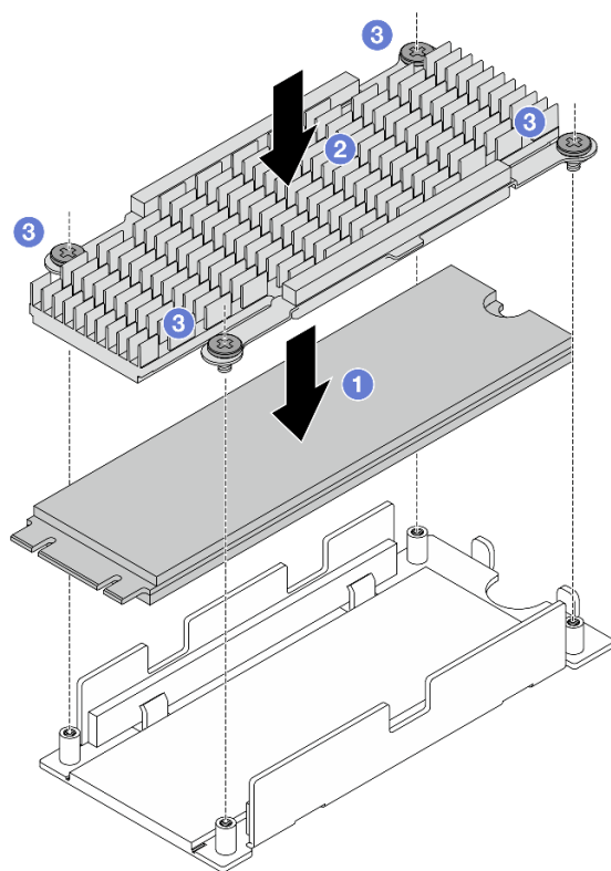
Abbildung 114. Installieren eines M.2-Laufwerks
