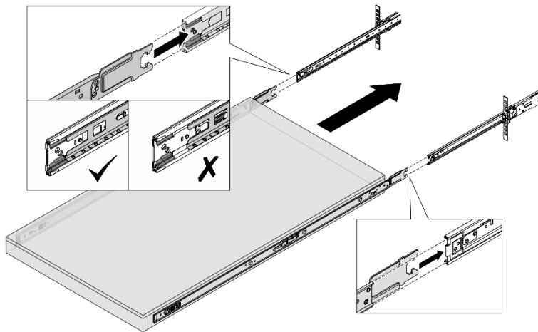
Abbildung 14. Verriegeln der Schienen
