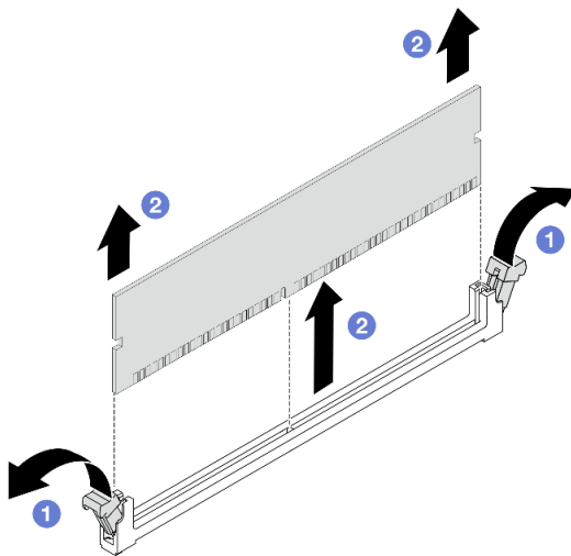
Abbildung 182. Entfernen des Speichermoduls
