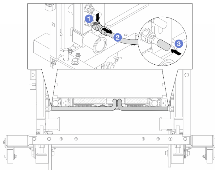
Abbildung 141. Entfernen der Schnellanschlüsse
