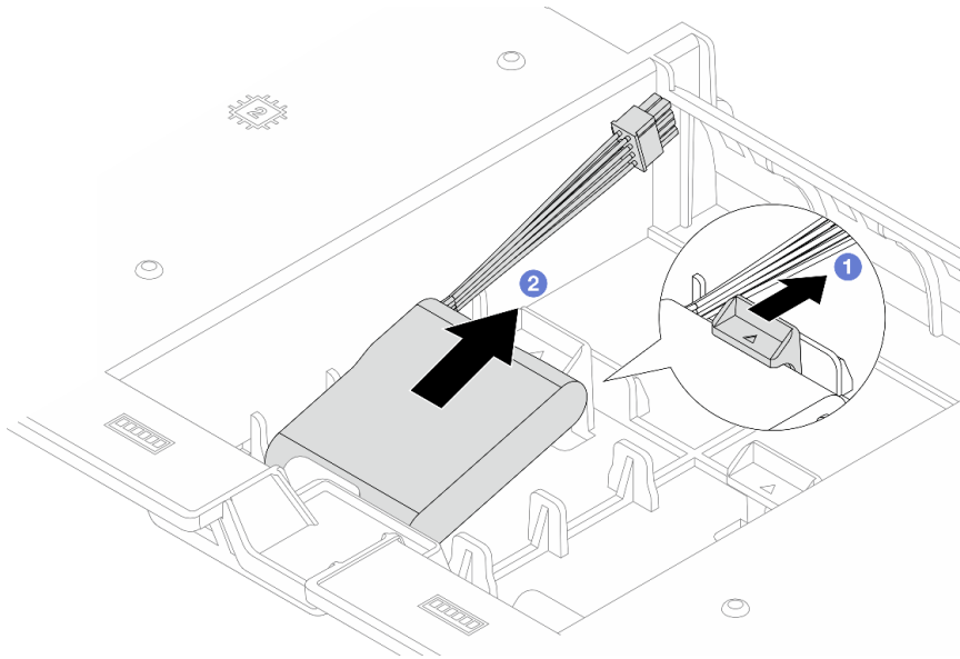
Abbildung 206. Entfernen des RAID-Flash-Stromversorgungsmoduls von der Luftführung
