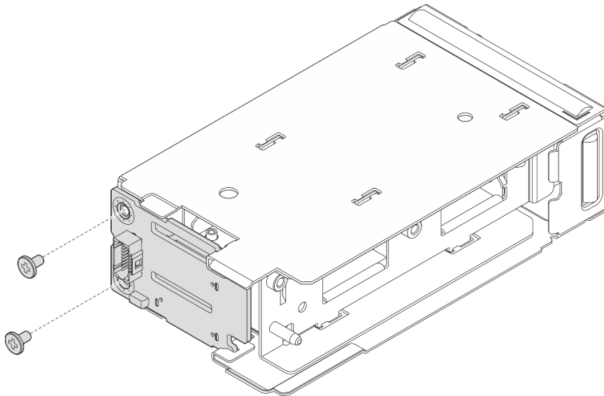
Abbildung 121. Entfernen der vorderen M.2-Boot-Rückwandplatine
