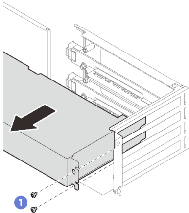
Abbildung 54. Entfernen des PCIe-Adapters
