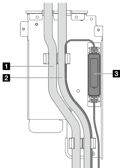
Abbildung 101. Installationsdetails
