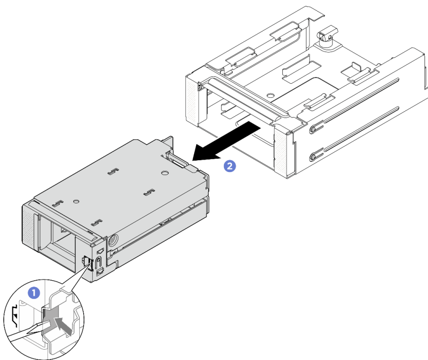
Abbildung 119. Entfernen der vorderen M.2-Laufwerkhalterung aus dem Rahmen
