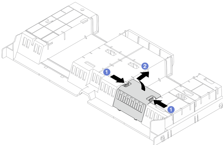
Abbildung 28. Entfernen der Abdeckblende der Luftführung
