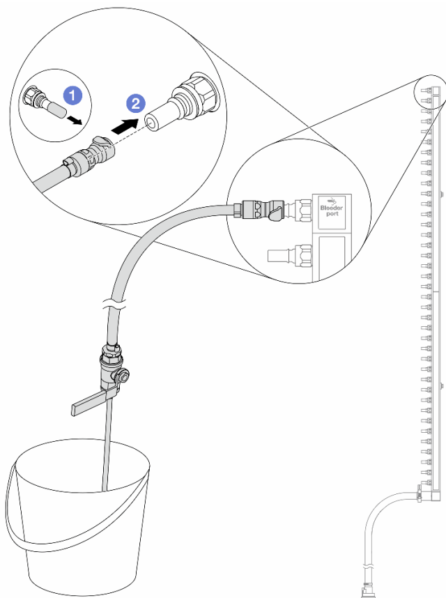
Abbildung 168. Installieren des Ablasssatzes an der Rücklaufseite
