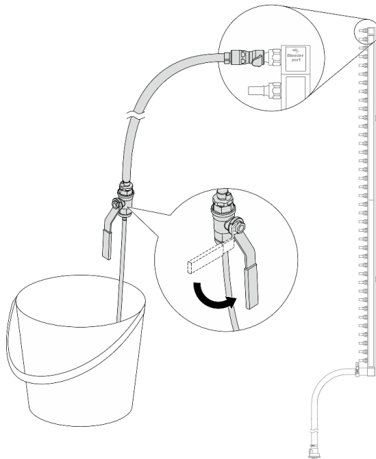
Abbildung 169. Öffnen des Ablassventils
