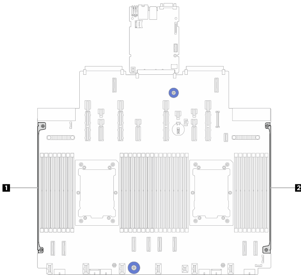
Abbildung 32. Positionen der Kabelwände
