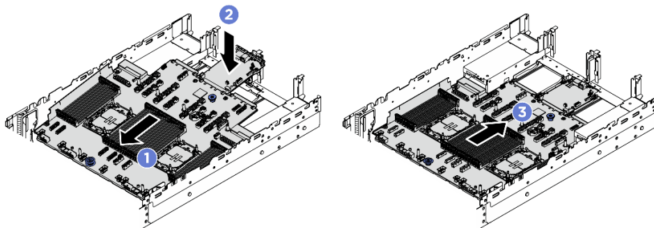
Abbildung 234. Installieren der Systemplatinenbaugruppe
