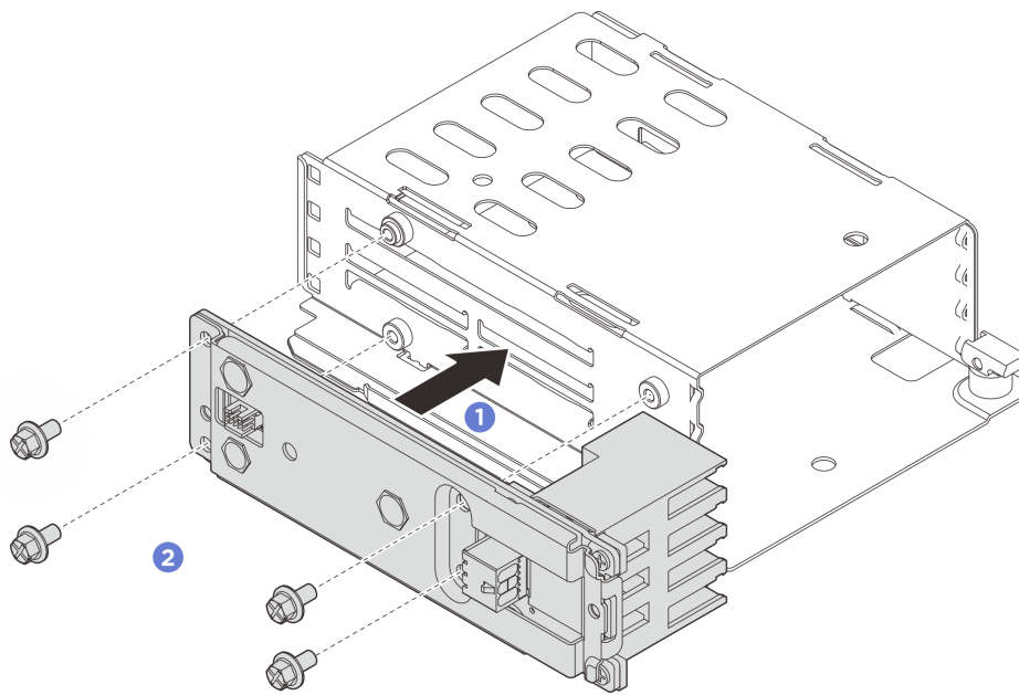
Abbildung 50. Installieren der Rückwandplatinenbaugruppe
