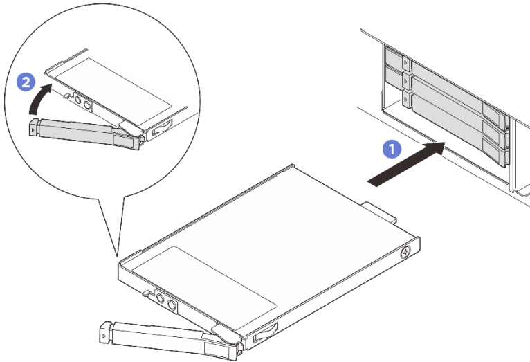
Abbildung 41. Installieren eines E3.S-Hot-Swap-Laufwerks
