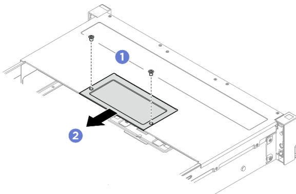
Abbildung 21. Entfernen der Abdeckplatte
