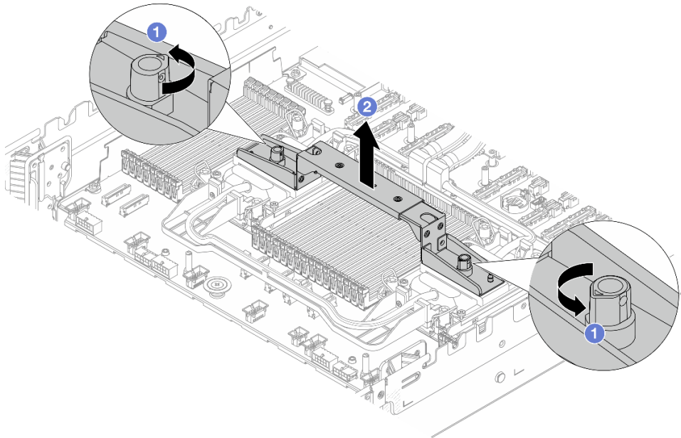
Abbildung 98. Entfernen des Modulgriffs
