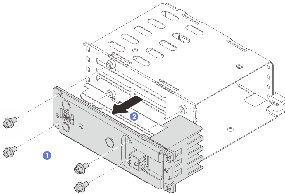
Abbildung 47. Entfernen der Rückwandplattenbaugruppe
