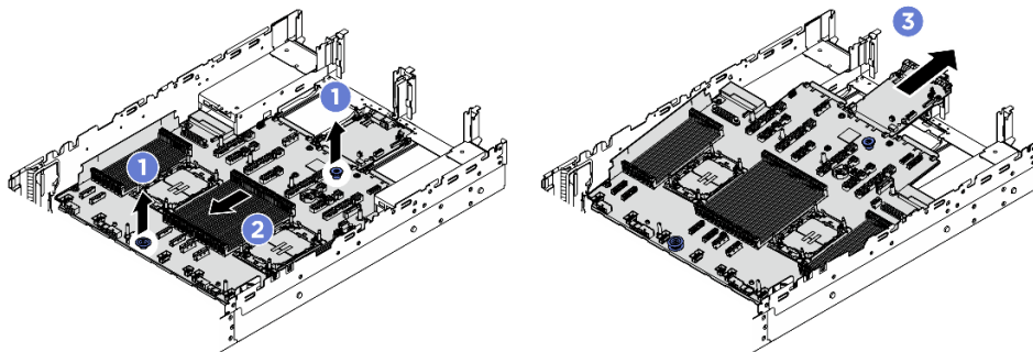
Abbildung 235. Entfernen der Systemplatinenbaugruppe
