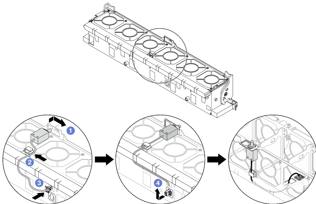
Abbildung 88. Installieren des Schalters gegen unbefugten Zugriff
