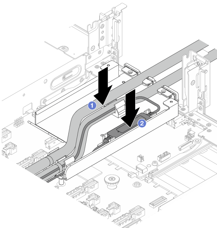
Abbildung 100. Platzieren der Schläuche und des Flüssigkeitserkennungssensormodul
