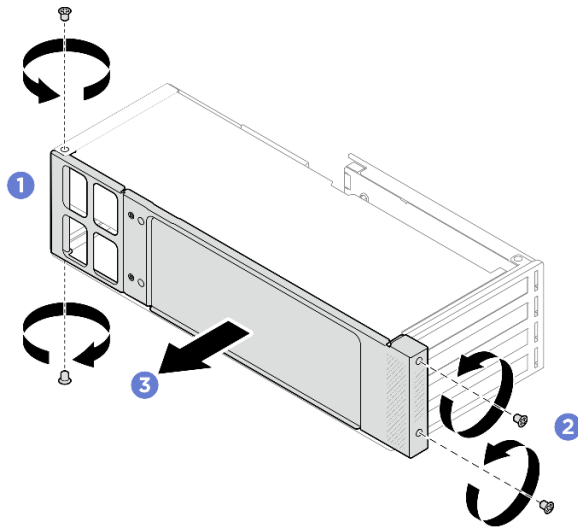
Abbildung 53. Entfernen der seitlichen Halterung
