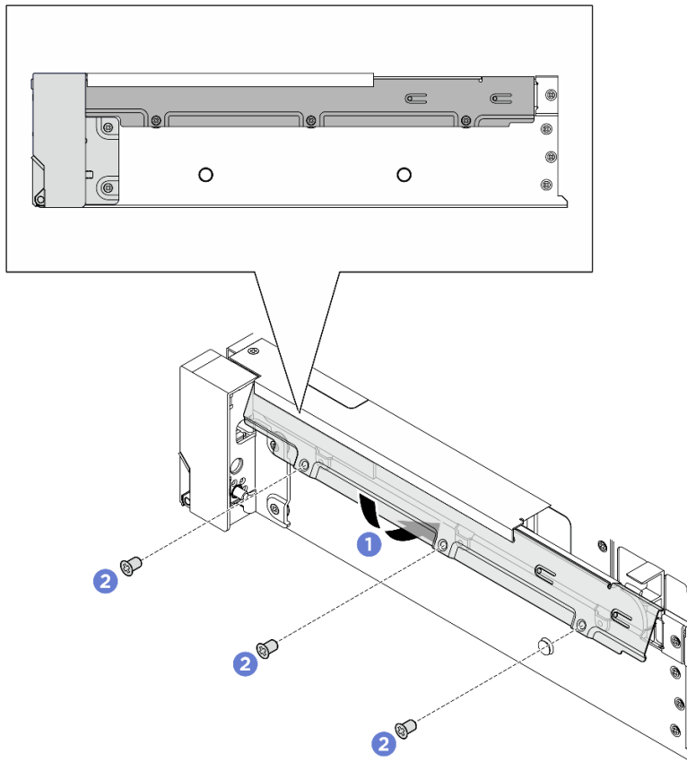
Abbildung 204. Anbringen der Kabelhalterung
