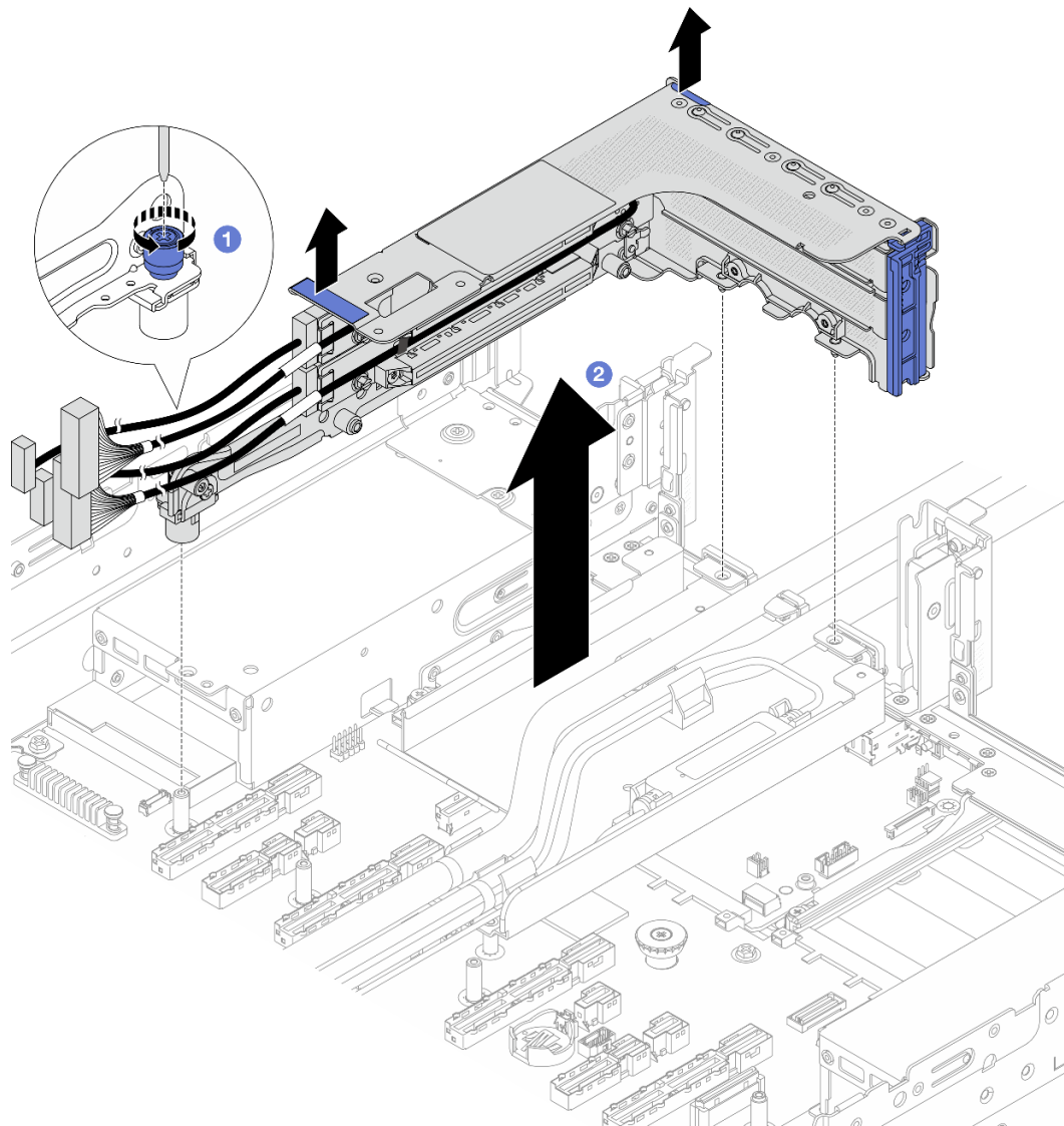
Abbildung 90. Entfernen des 3FH-Adapterrahmens
