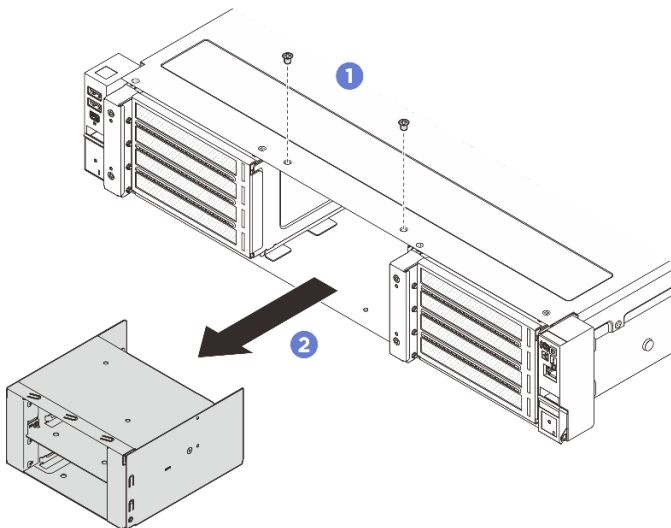
Abbildung 48. Entfernen der E3.S-Laufwerkhalterung
