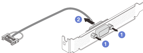
Abbildung 226. Zerlegen des seriellen Anschlussmoduls
