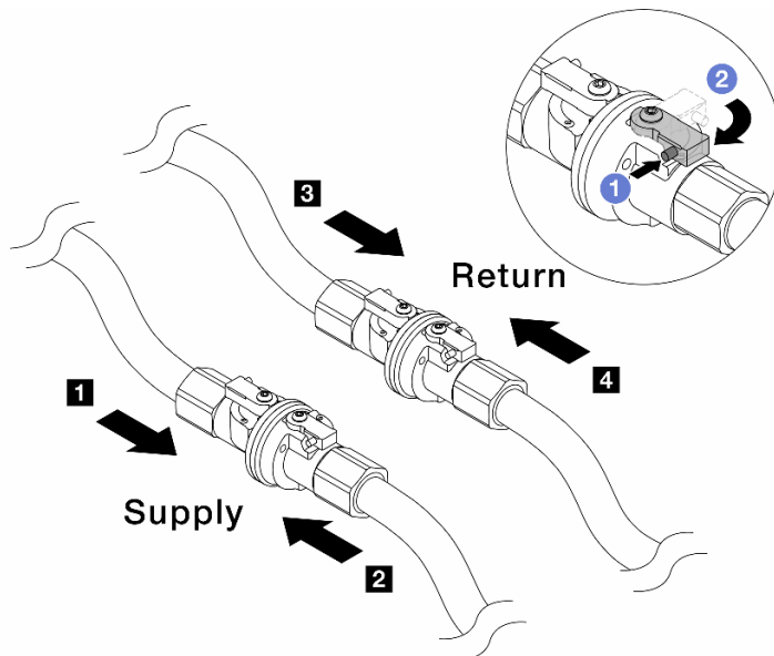
Abbildung 181. Öffnen der Kugelhähne
