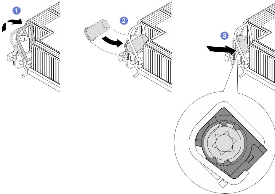
Abbildung 66. Anbringen einer T30-Torx-Mutter am Kühlkörper
