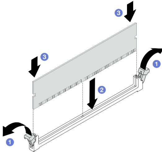
Abbildung 183. Installieren des Speichermoduls
