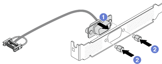
Abbildung 227. Montieren des seriellen Anschlussmoduls
