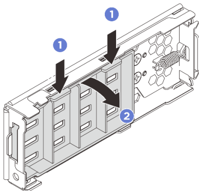
Abbildung 43. Entfernen der inneren Platte
