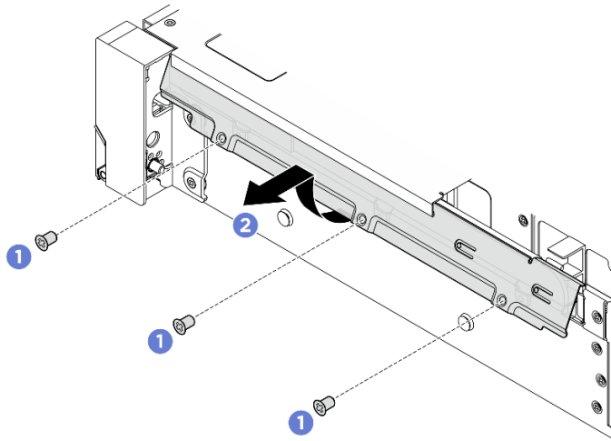
Abbildung 199. Entfernen der Kabelhalterung
