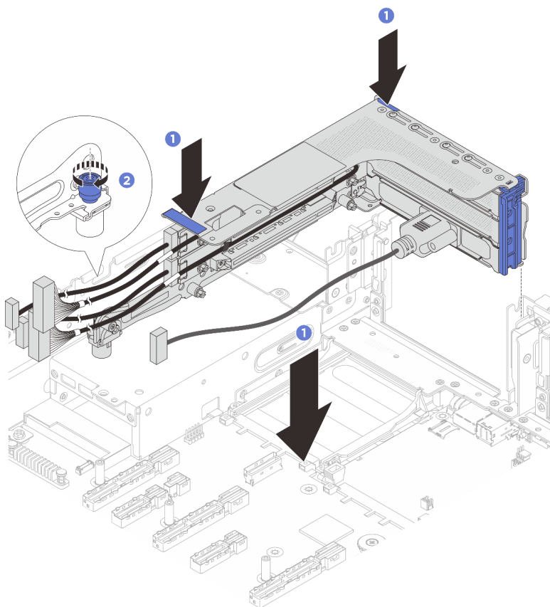
Abbildung 229. Installieren der Adapterkartenbaugruppe
