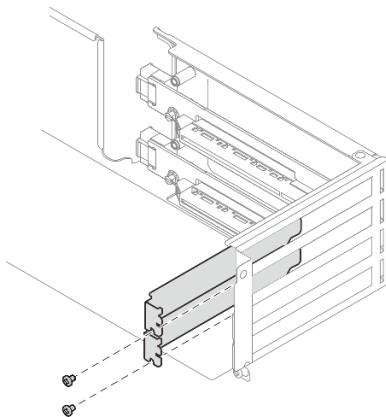
Abbildung 55. Abdeckblende für PCIe-Steckplatz
