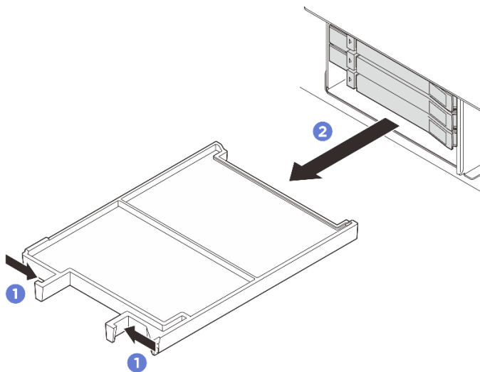
Abbildung 40. Entfernen einer Abdeckblende für die Position
