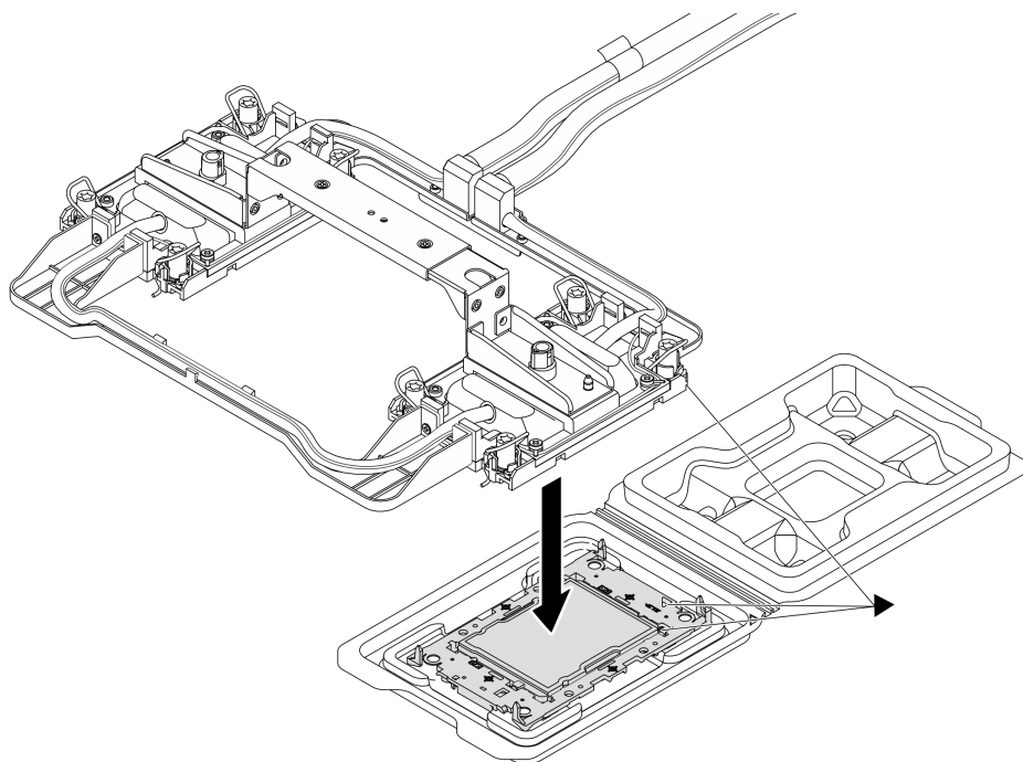
Abbildung 95. Installieren des Prozessors
