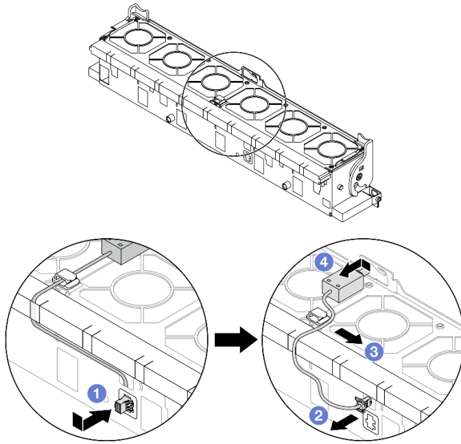
Abbildung 87. Entfernen des Schalters gegen unbefugten Zugriff
