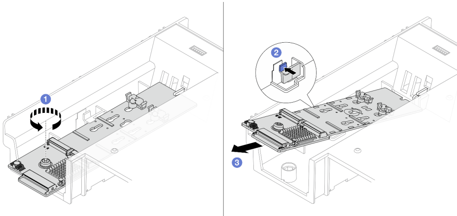
Abbildung 83. Entfernen der M.2-Rückwandplatine von der Luftführung
