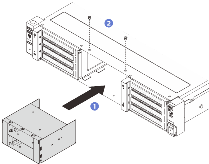
Abbildung 49. Installieren der E3.S-Halterung
