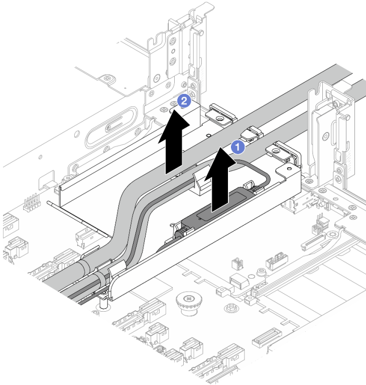
Abbildung 91. Trennen der Schläuche und Flüssigkeitserkennungssensormodul
