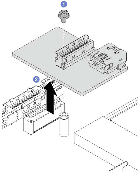
Abbildung 246. Entfernen der USB-E/A-Platine
