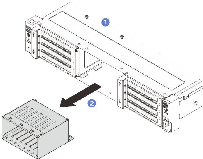
Abbildung 23. Entfernen der 2,5-Zoll-Laufwerkhalterung
