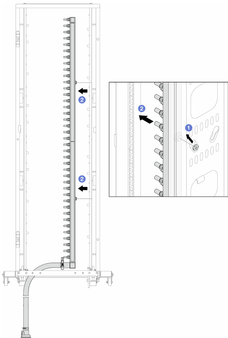
Abbildung 165. Entfernen der Leitung
