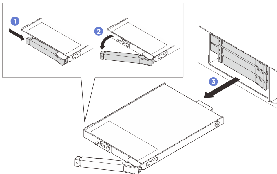
Abbildung 38. Entfernen eines E3.S-Hot-Swap-Laufwerks
