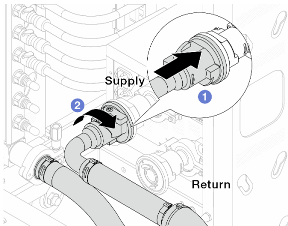
Abbildung 153. Verbinden der Kugelhähne
