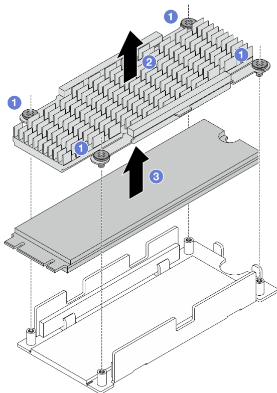
Abbildung 111. Entfernen eines M.2-Laufwerks
