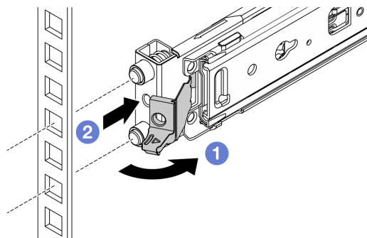
Abbildung 3. Entfernen der Schiene an der Vorderseite
