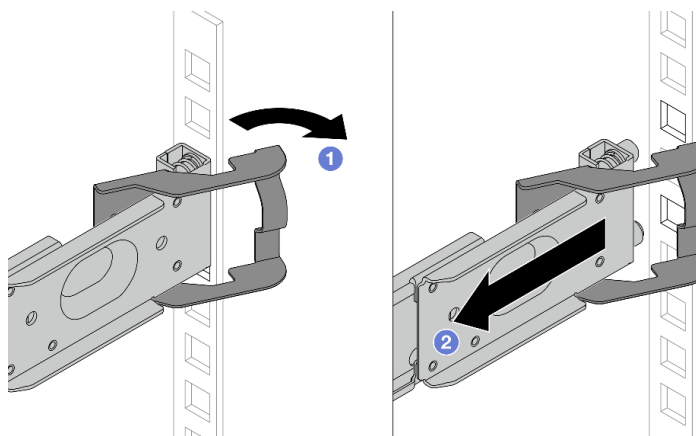
Abbildung 4. Entfernen der Schiene an der Rückseite
