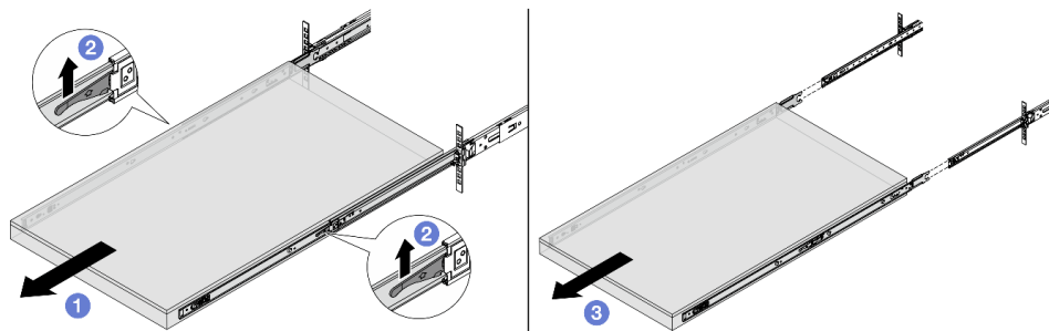
Abbildung 9. Herausziehen des Servers
