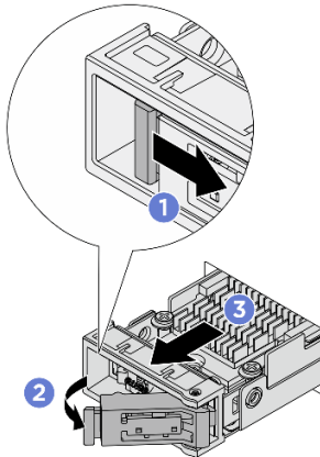
Abbildung 105. Entfernen einer Hot-Swap-M.2-Laufwerkbaugruppe
