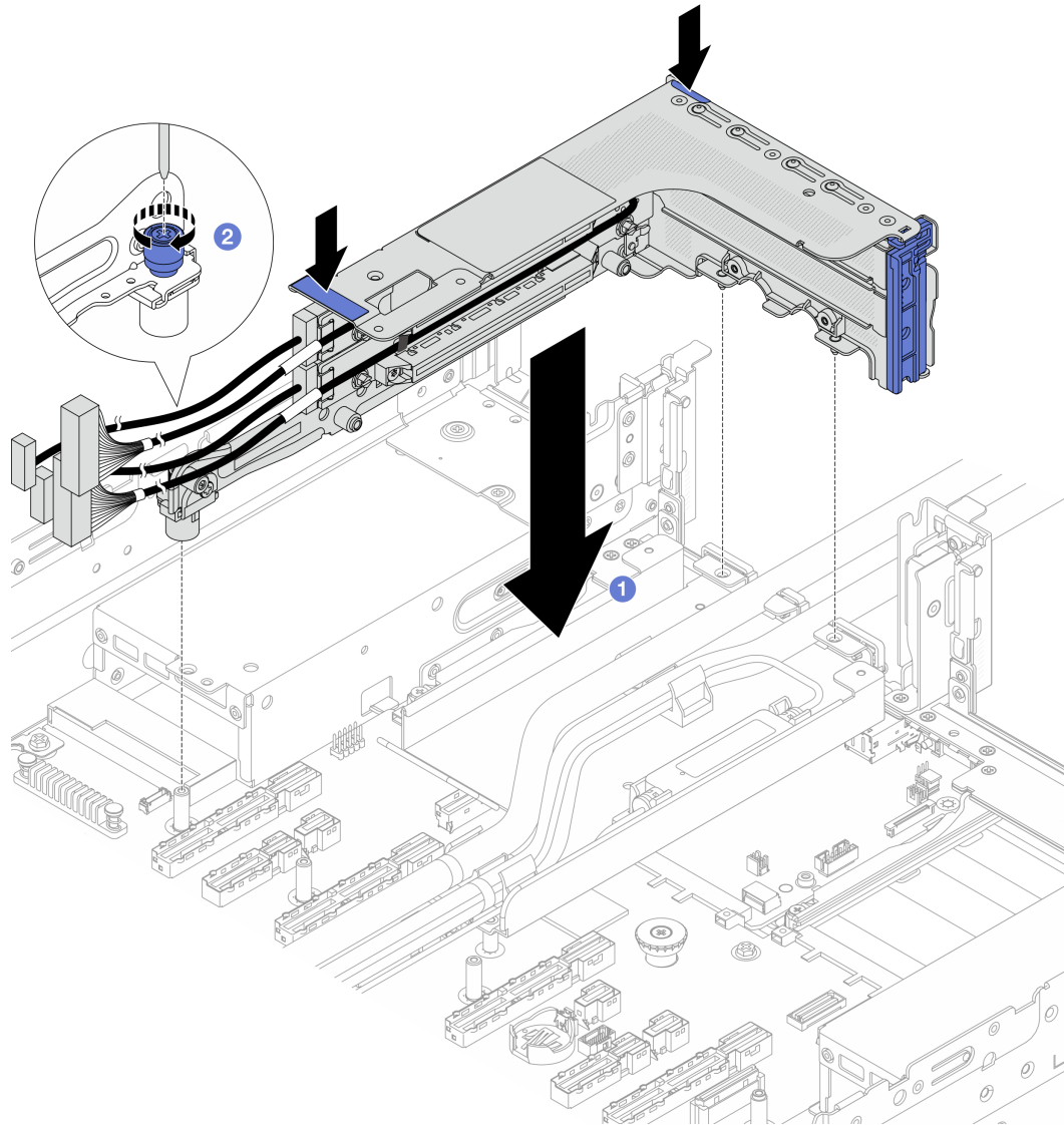
Abbildung 103. Installieren des 3FH-Adapterrahmens
