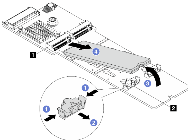
Abbildung 78. M.2-Laufwerk entfernen
