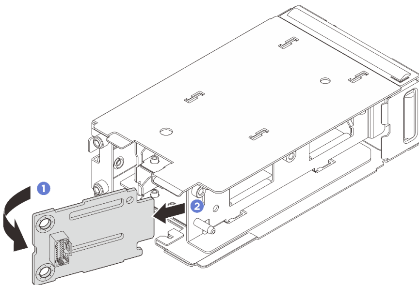
Abbildung 122. Entfernen der vorderen M.2-Boot-Rückwandplatine
