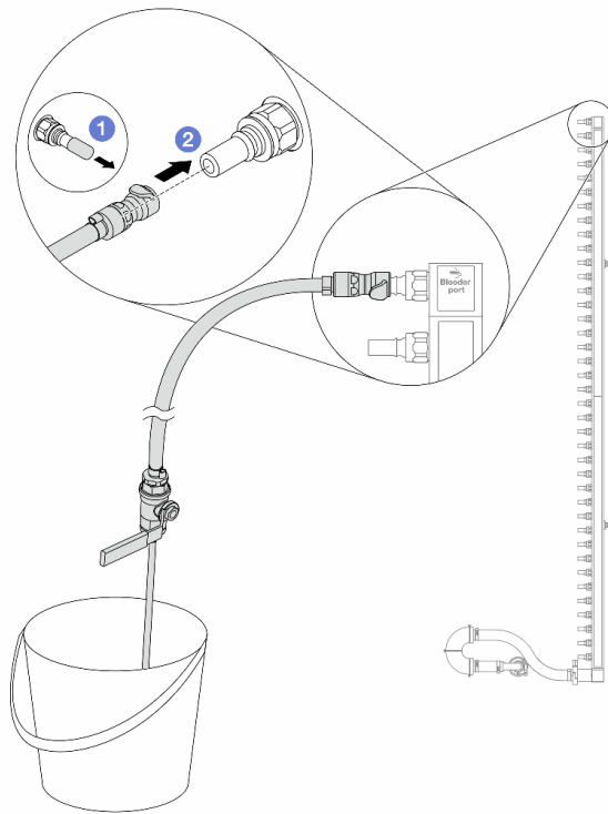
Abbildung 146. Installieren des Ablasssatzes an der Rücklaufseite
