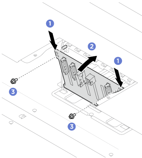
Abbildung 25. Installieren der Rückwandplatine für 2,5-Zoll-Laufwerke
