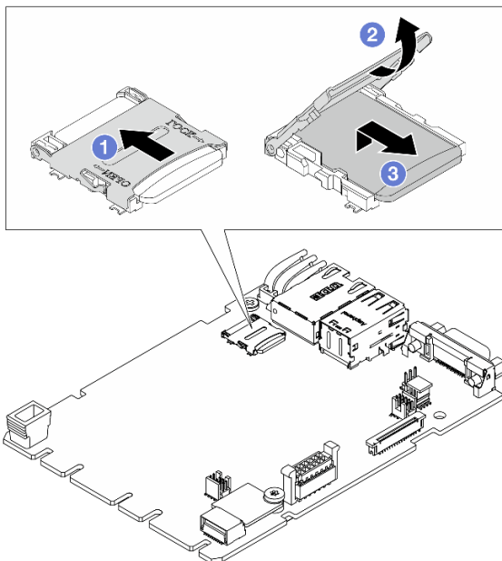
Abbildung 184. Entfernen der microSD-Karte
