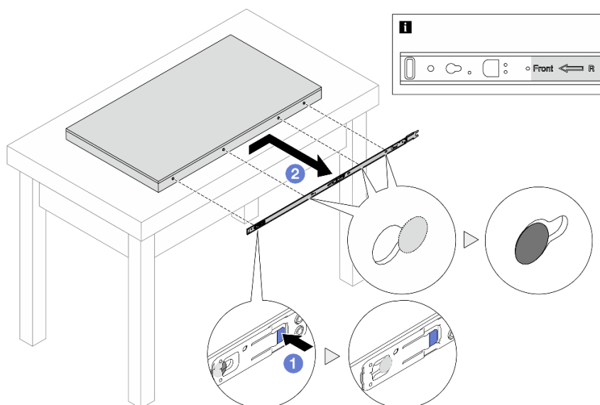
Abbildung 10. Entfernen der inneren Schienen
