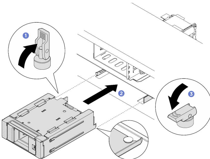
Abbildung 128. Installieren der vorderen M.2-Laufwerkhalterung mit Rahmen
