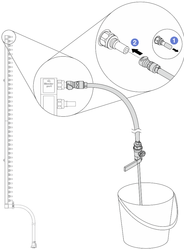
Abbildung 166. Installieren des Ablasssatzes an der Zulaufseite
