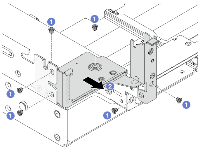
Abbildung 218. Entfernen der linken Rückwandhalterung
