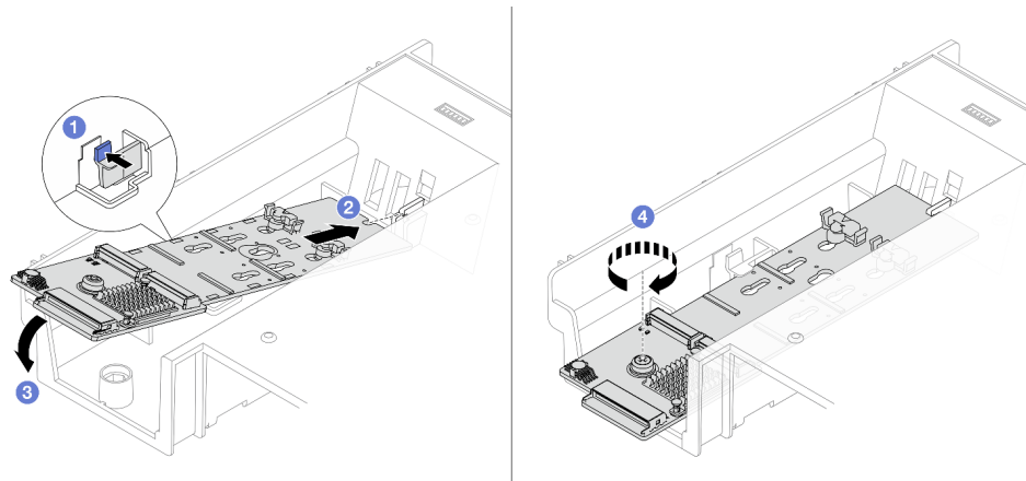
Abbildung 84. Installieren der M.2-Rückwandplatine an der Luftführung
