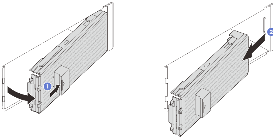
Abbildung 37. Entfernen der E3.S-Blende
