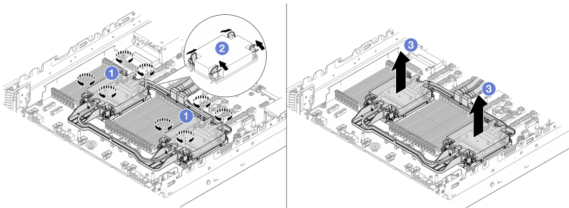
Abbildung 92. Entfernen der Processor Neptune Core Module
