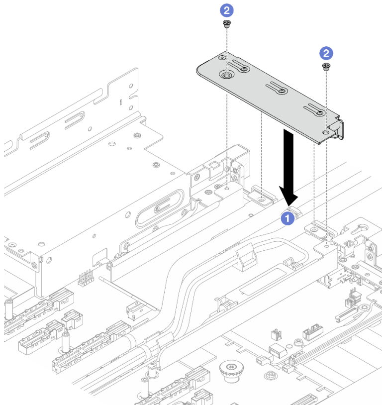
Abbildung 102. Installieren der 1FH-Halterung
