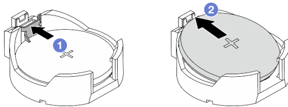
Abbildung 35. Entfernen der CMOS-Batterie
