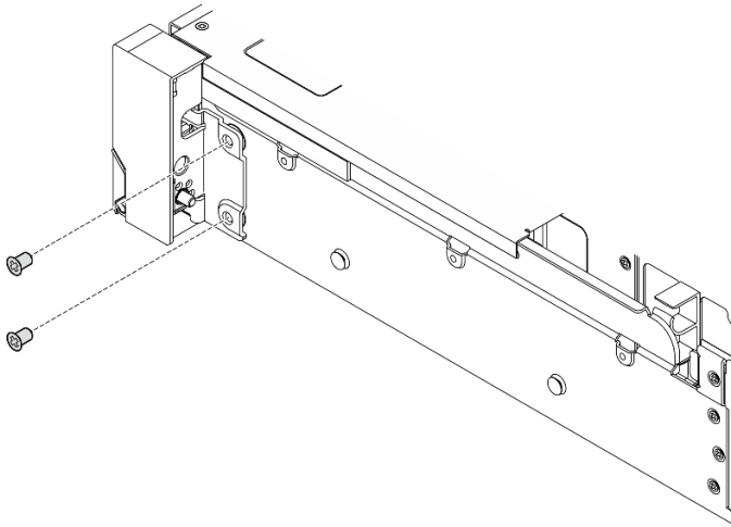
Abbildung 203. Installieren der Schrauben
