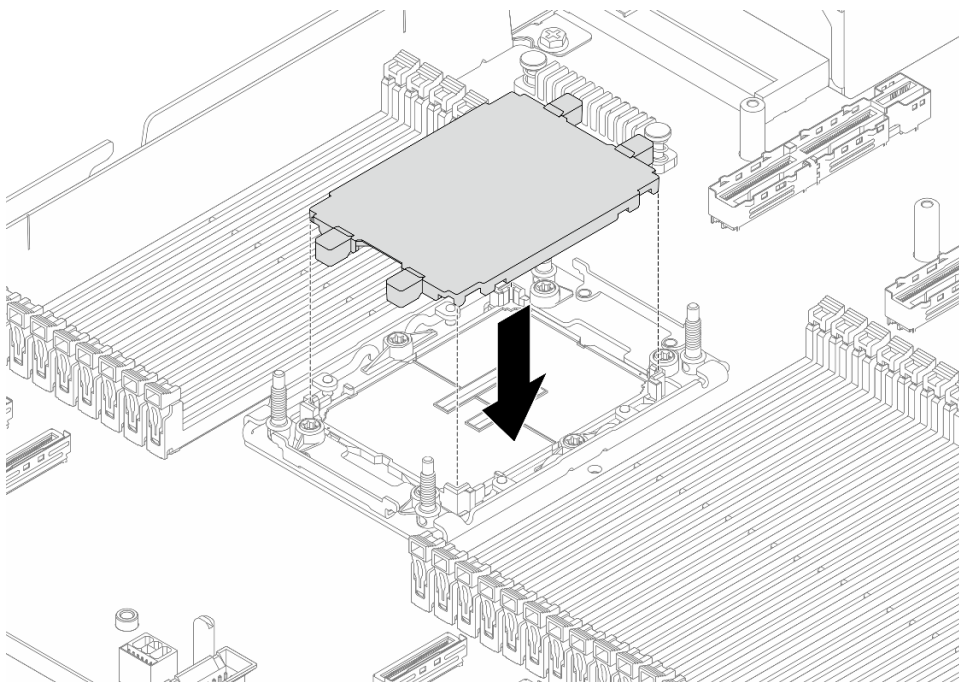
Abbildung 96. Installieren der Prozessorsockelabdeckung
