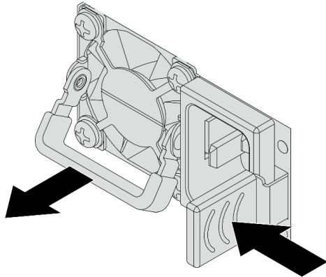
Abbildung 69. Entfernen der Hot-Swap-Netzteilereinheit
