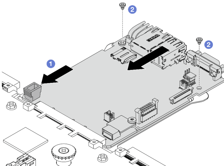
Abbildung 237. Installieren der System-E/A-Platine auf der Prozessorplatine
