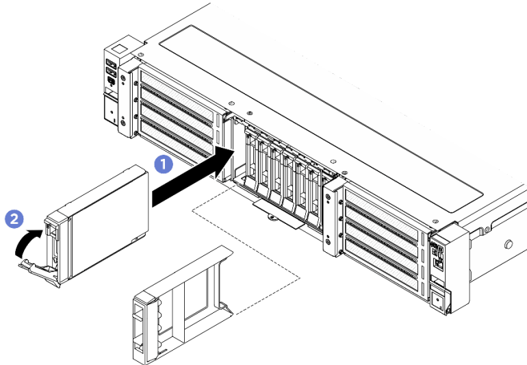
Abbildung 20. Installieren eines 2,5-Zoll-Hot-Swap-Laufwerks
