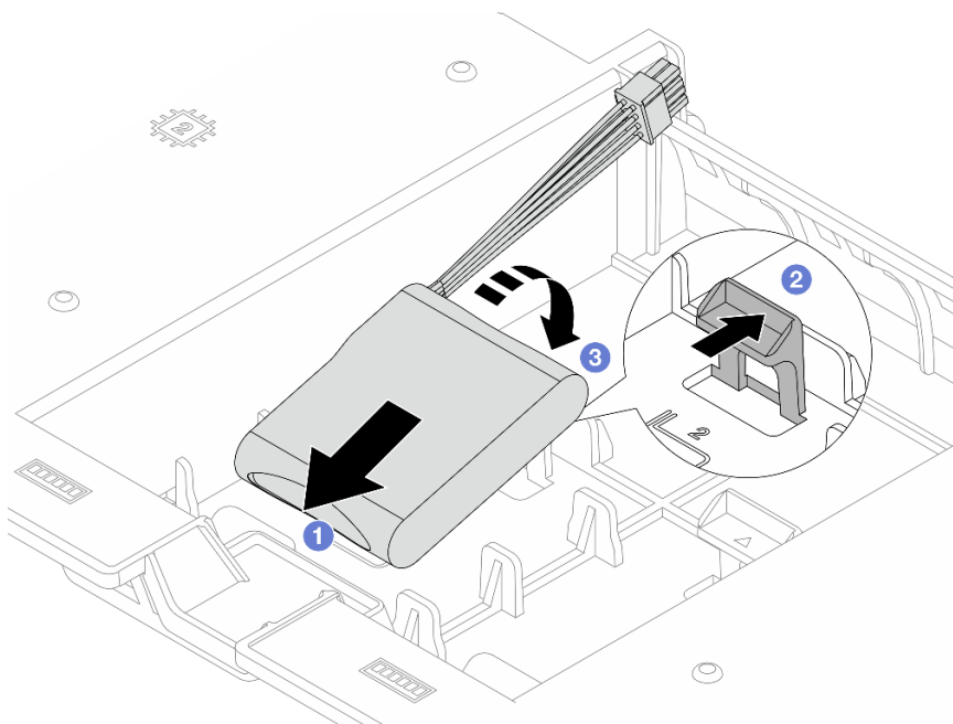
Abbildung 207. Installieren des RAID-Flash-Stromversorgungsmoduls an der Luftführung
