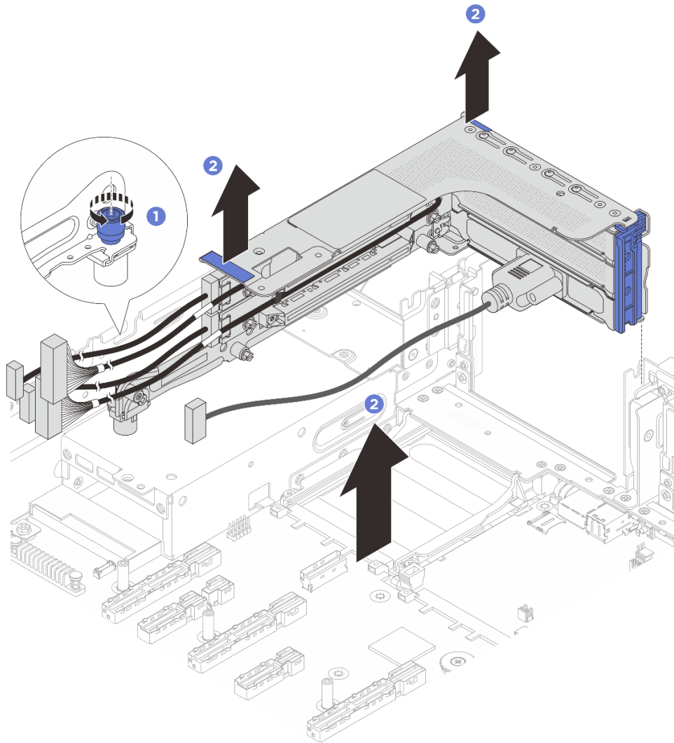
Abbildung 224. Adapterkartenbaugruppe entfernen
