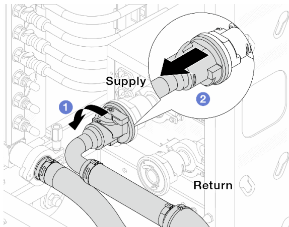
Abbildung 142. Entfernen des Verbindungssatzes
