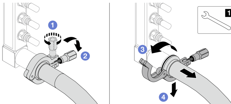
Abbildung 170. Trennen der Leitung vom Schlauchsatz
