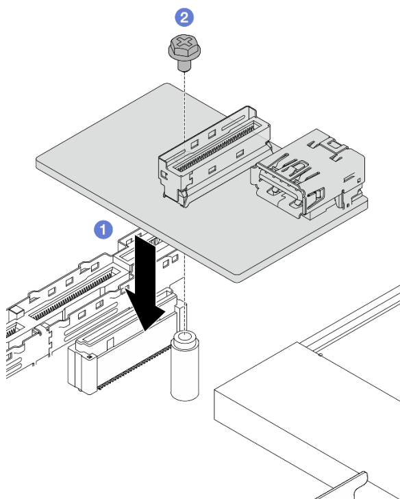
Abbildung 247. Installieren der USB-E/A-Platine
