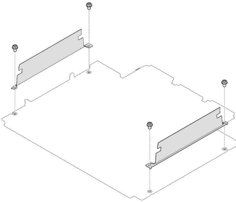
Abbildung 33. Entfernen der Kabelwände
