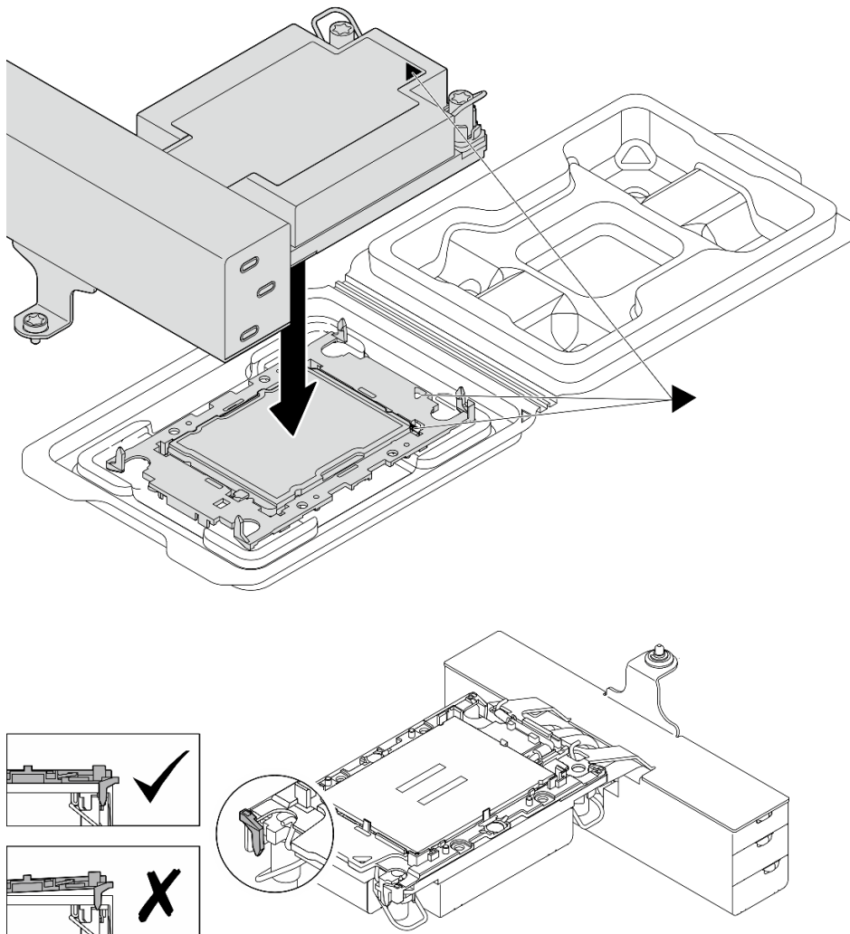
Abbildung 195. Zusammenbauen der PHM mit Prozessor im Versandeinbaurahmen
