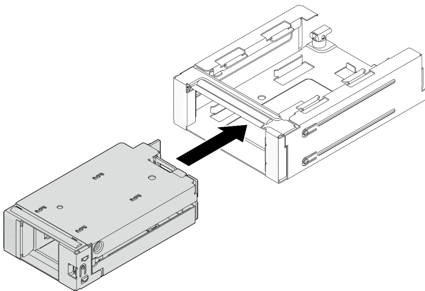
Abbildung 127. Installieren der vorderen M.2-Laufwerkhalterung im Rahmen
