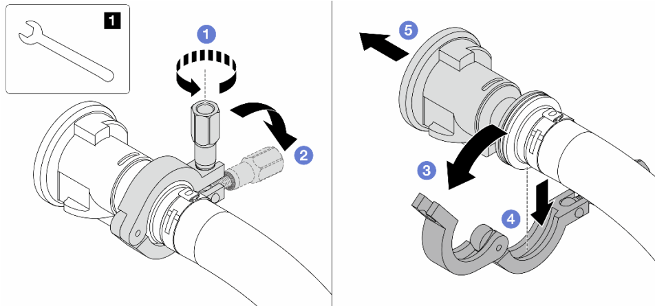
Abbildung 150. Trennen der Kugelhähne
