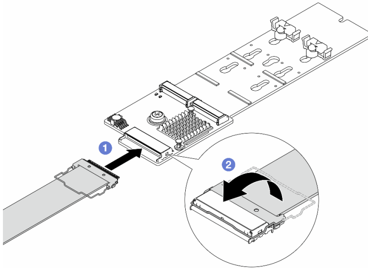
Abbildung 85. Verbinden des M.2-Kabels
