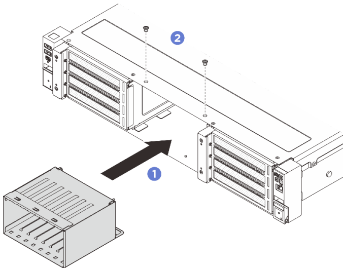
Abbildung 24. Installieren der 2,5-Zoll-Laufwerkhalterung
