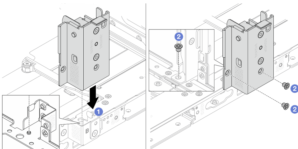
Abbildung 222. Installieren der mittleren Rückwandhalterung
