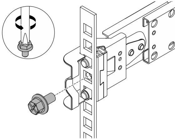
Abbildung 2. Entfernen der M6-Schrauben
