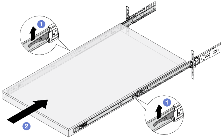
Abbildung 15. Verriegeln der Schienen und Einschieben in den Server
