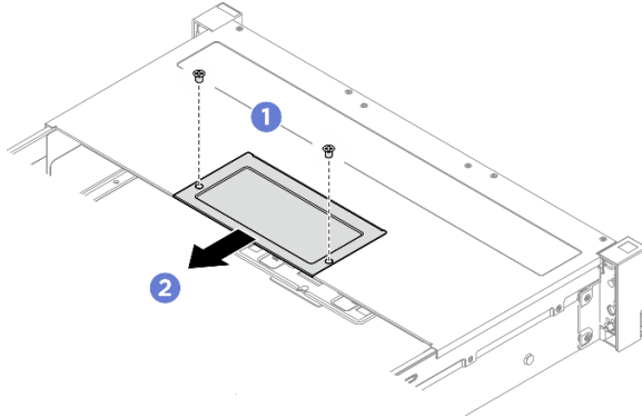
Abbildung 75. Entfernen der Abdeckplatte
