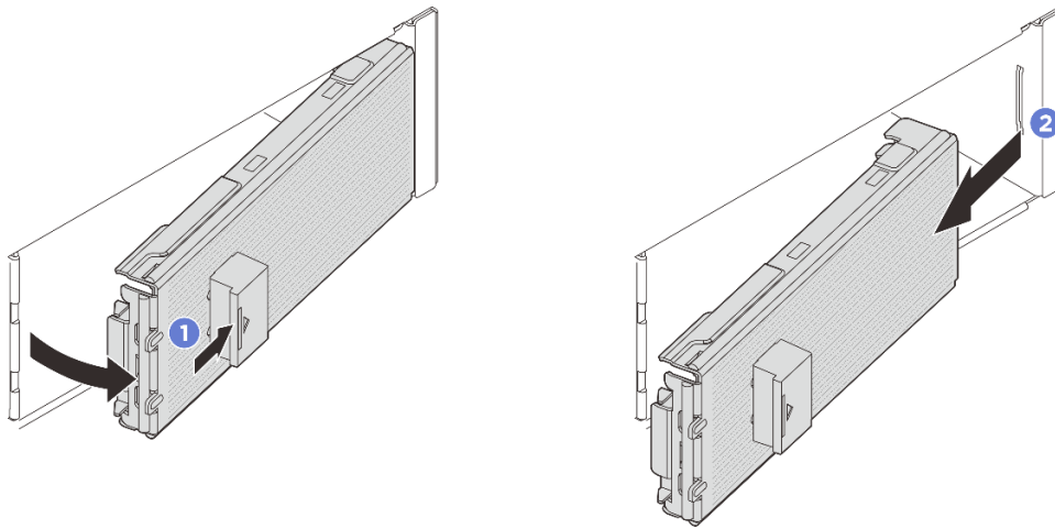
Abbildung 39. Entfernen der E3.S-Blende
