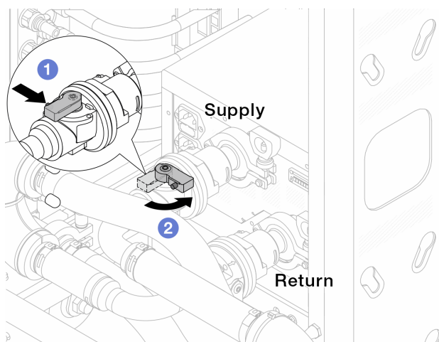
Abbildung 140. Schließen der Kugelhähne
