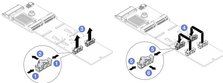
Abbildung 79. M.2-Halterung anpassen
