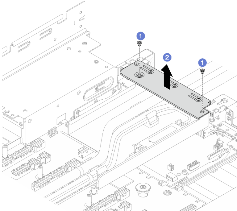
Abbildung 89. Entfernen der 1FH-Halterung
