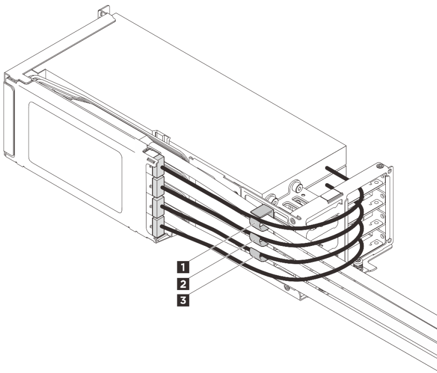
Abbildung 58. Kabelklemmen der Adapterkartenbaugruppe an der Vorderseite
