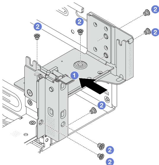
Abbildung 223. Installieren der rechten Rückwandhalterung
