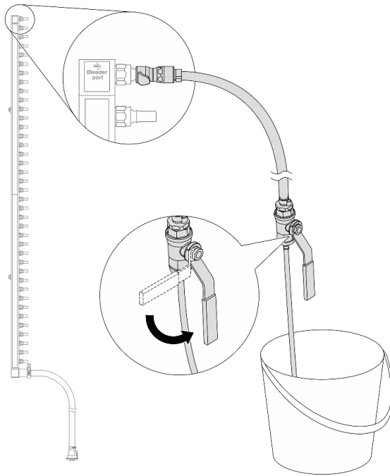
Abbildung 167. Öffnen des Ablassventils
