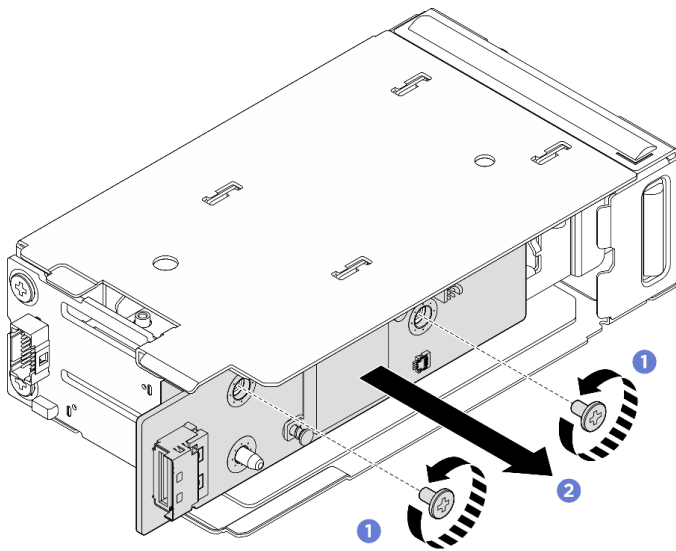
Abbildung 120. Entfernen der vorderen M.2-Controllerplatine
