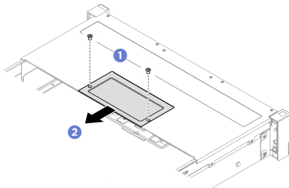
Abbildung 45. Entfernen der Abdeckplatte
