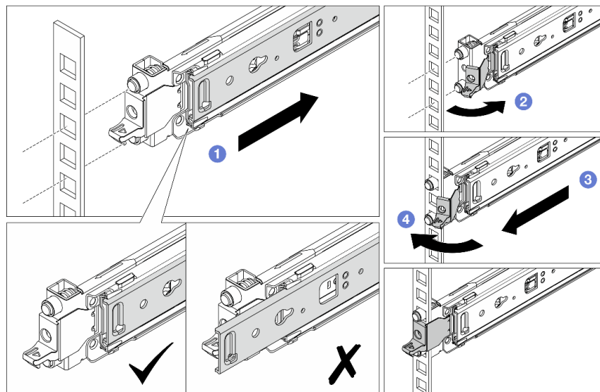
Abbildung 6. Installieren der vorderen Befestigungsstifte
