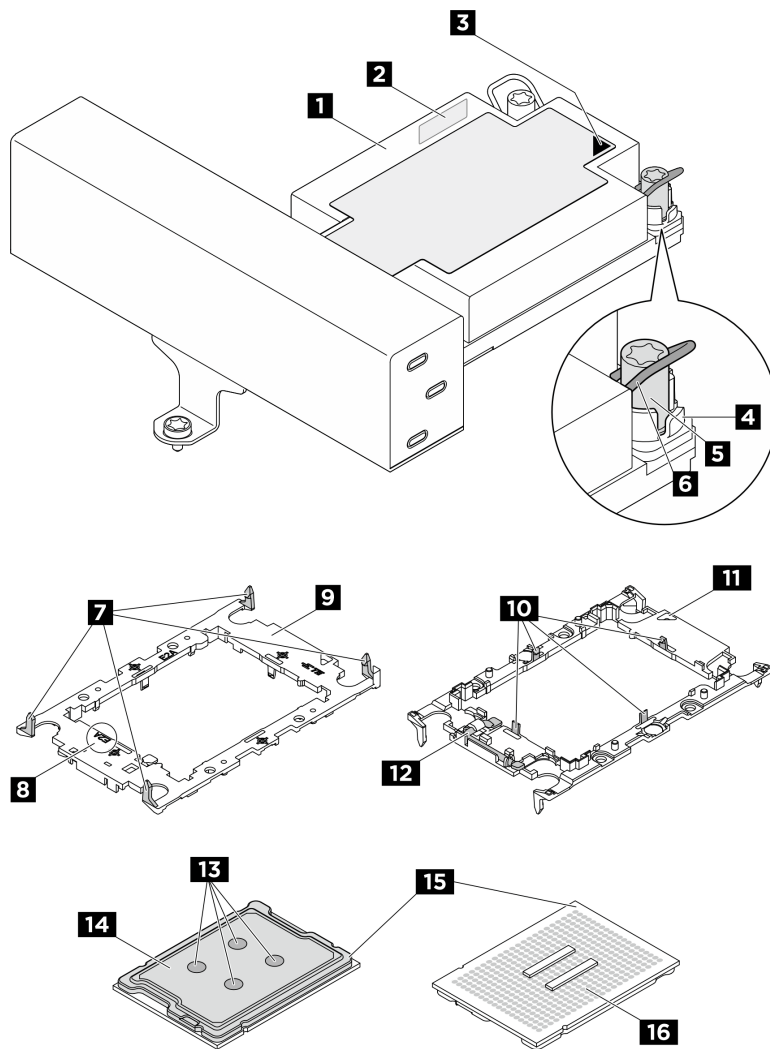
Abbildung 192. PHM-Komponenten
