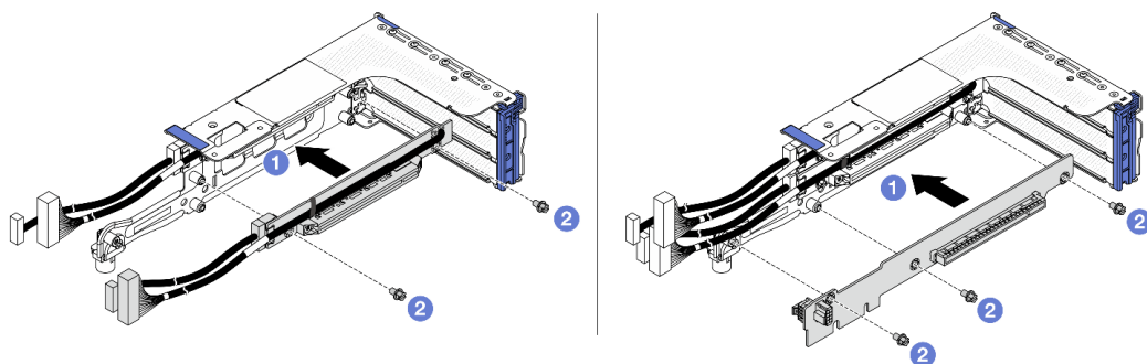
Abbildung 215. Installieren der Adapterkarten im 3FH-Adapterrahmen
