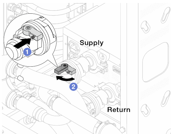
Abbildung 158. Öffnen der Kugelhähne
