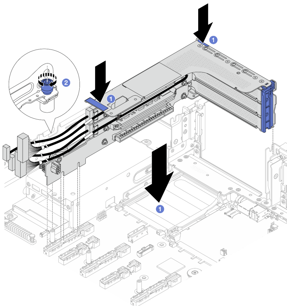
Abbildung 217. Installieren der 3FH-Adapterkartenbaugruppe
