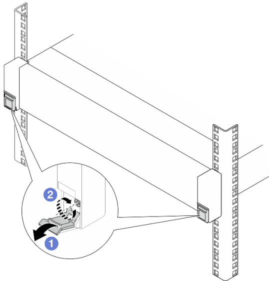
Abbildung 16. Sichern des Servers an der Vorderseite des Racks
