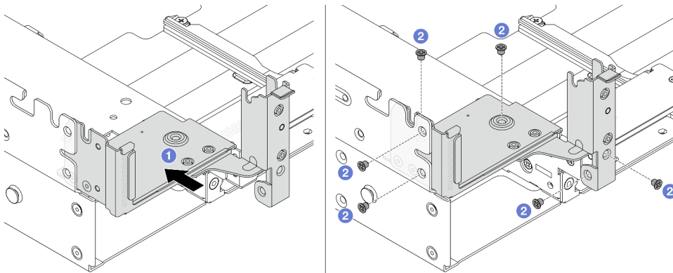
Abbildung 221. Installieren der linken Rückwandhalterung
