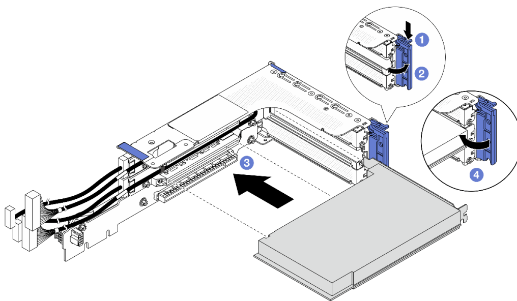
Abbildung 216. Installieren eines PCIe-Adapters im 3FH-Adapterrahmen
