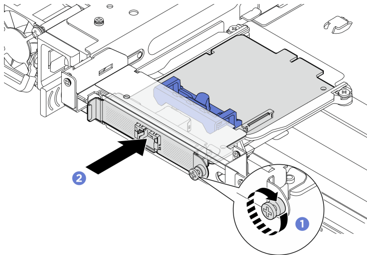
Abbildung 133. Installieren des NIC-Verwaltungsadapters
