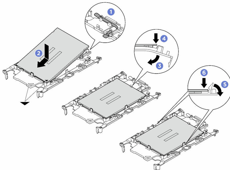
Abbildung 193. Installieren eines Prozessorträgers
