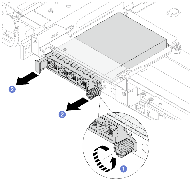
Abbildung 208. Herausnehmen des hinteren OCP-Moduls
