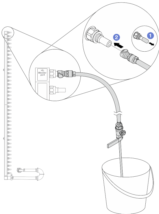
Abbildung 144. Installieren des Ablasssatzes an der Zulaufseite
