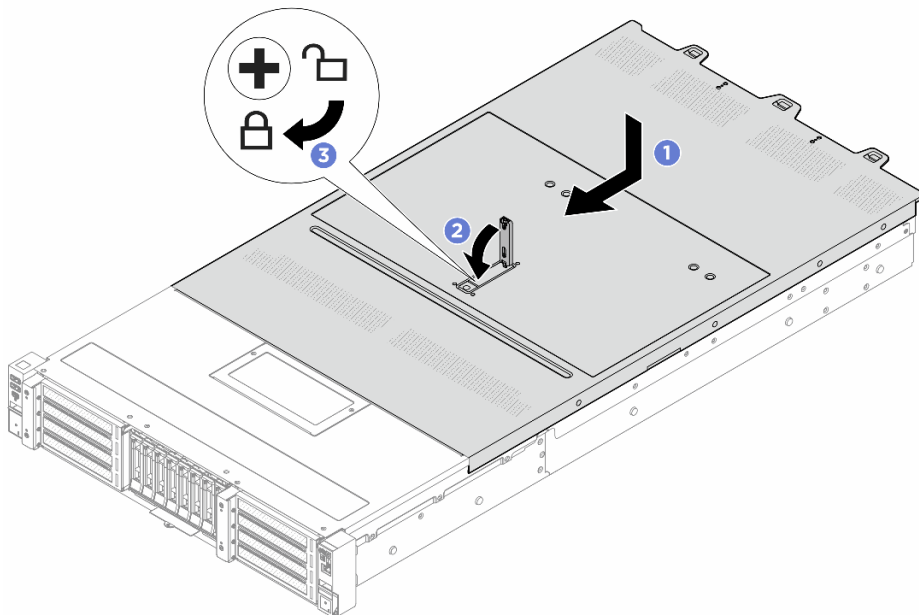
Abbildung 245. Installieren der oberen Abdeckung
