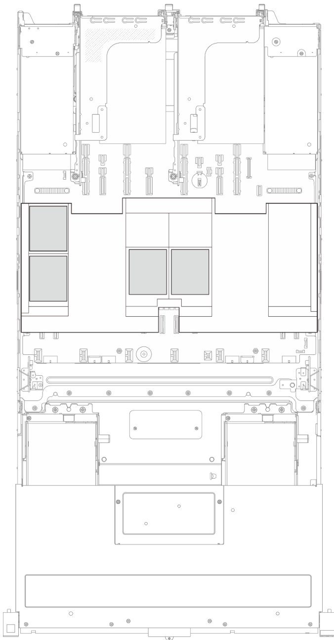
Abbildung 205. Position des RAID-Flashstromversorgungsmoduls an der Luftführung
