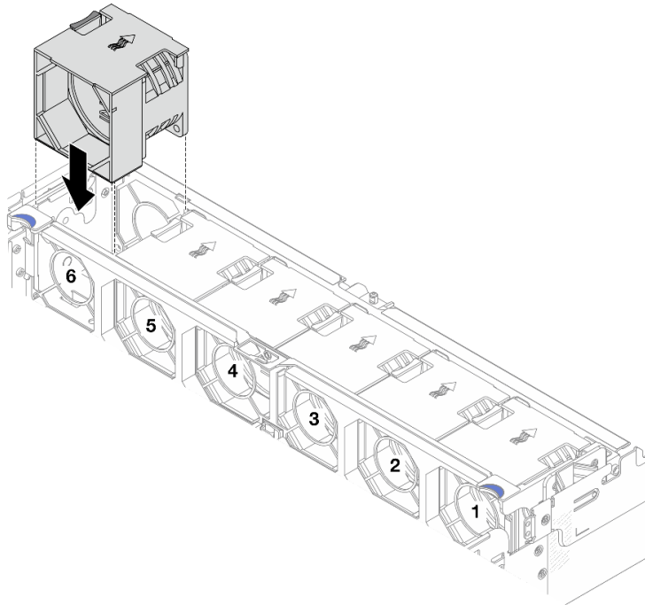
Abbildung 240. Installieren des Systemlüfters
