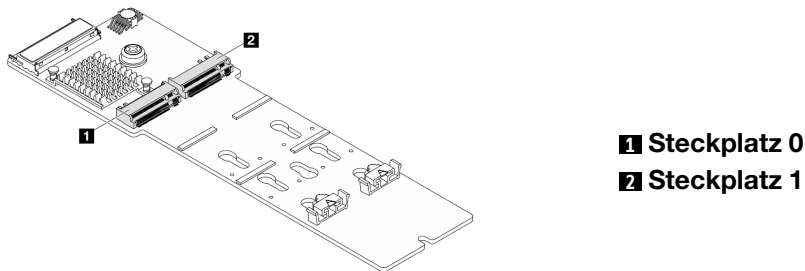
Abbildung 80. M.2-Laufwerksteckplätze
