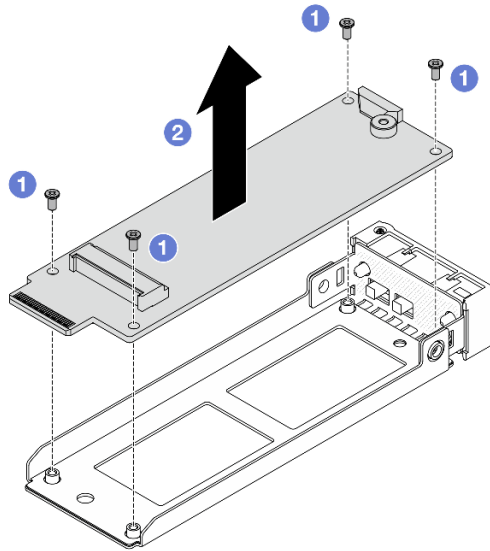
Abbildung 110. Entfernen des M.2-Interposers
