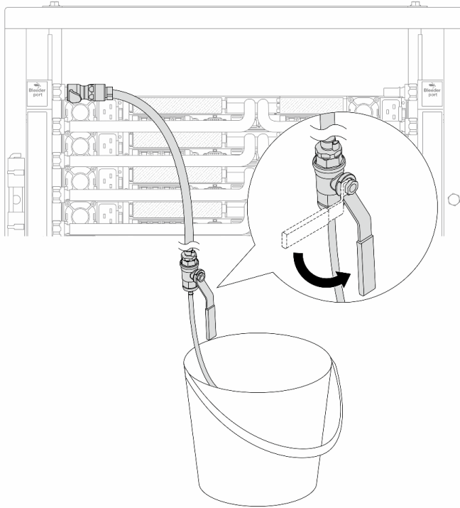
Abbildung 162. Öffnen des Ablassventils an der Zulaufseite
