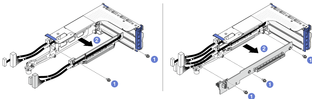
Abbildung 214. Entfernen der Adapterkarten aus dem Adapterrahmen
