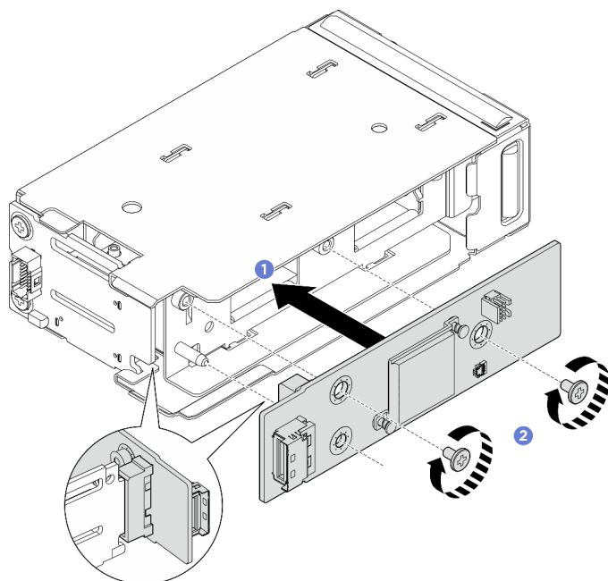
Abbildung 126. Installieren der vorderen M.2-Controllerplatine
