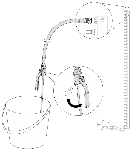
Abbildung 147. Öffnen des Ablassventils
