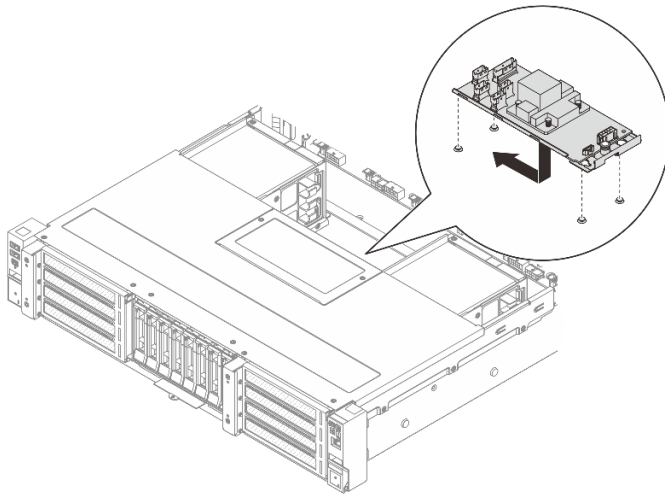
Abbildung 77. Installieren des internen CFF-Adapters
