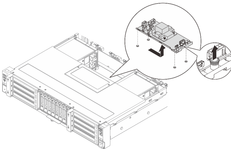
Abbildung 76. Entfernen des internen CFF-Adapters
