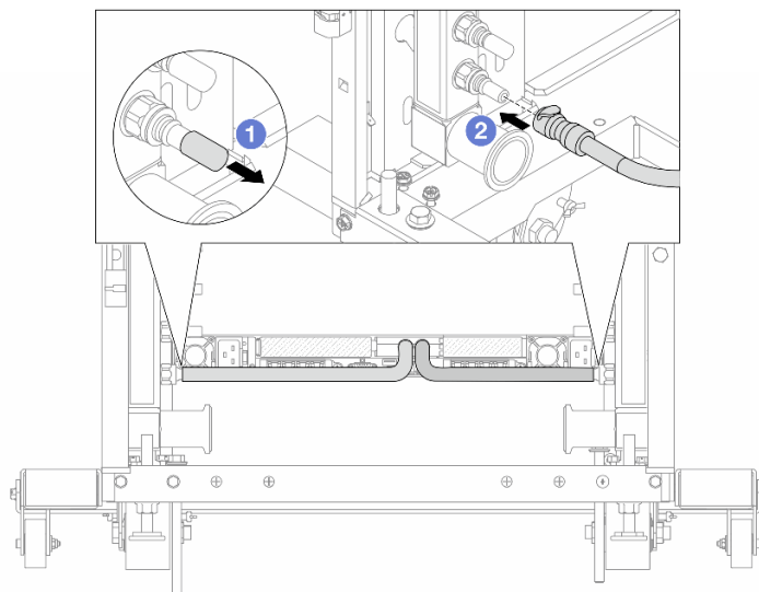
Abbildung 156. Anbringen der Schnellanschlüsse
