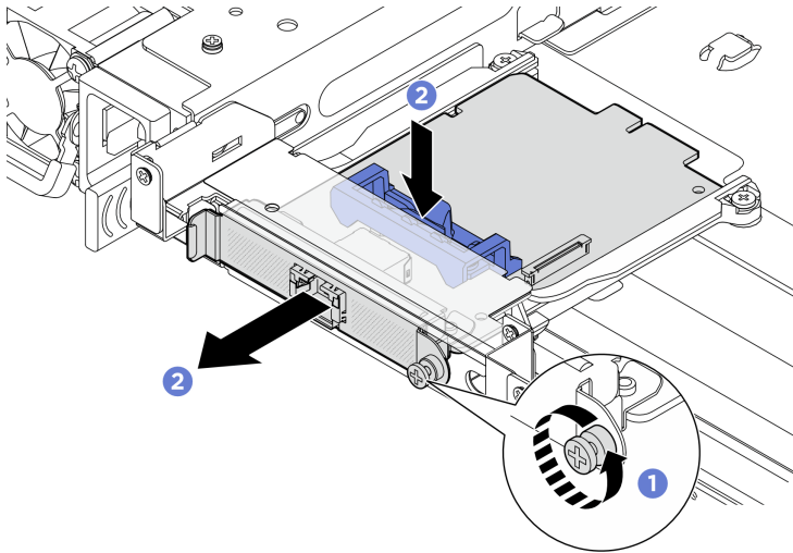
Abbildung 132. Entfernen des NIC-Verwaltungsadapters
