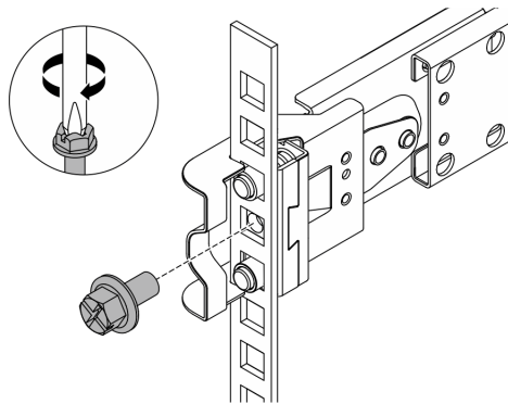
Abbildung 17. Sichern des Servers an der Rückseite des Racks
