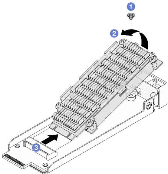
Abbildung 109. M.2-Laufwerk mit Kühlkörper entfernen
