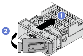
Abbildung 108. Installieren einer M.2-Laufwerkbaugruppe
