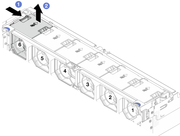
Abbildung 239. Systemlüfter entfernen
