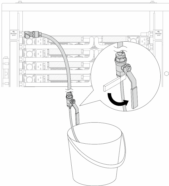
Abbildung 159. Öffnen des Ablassventils an der Zulaufseite
