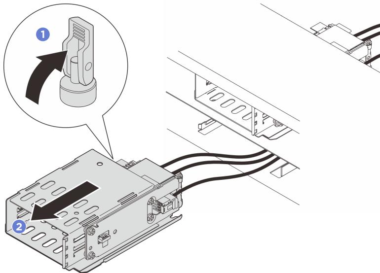
Abbildung 46. Entfernen der E3.S-1T-Halterung
