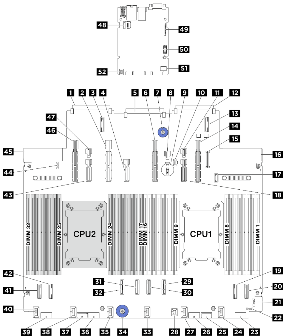
Abbildung 9. Anschlüsse auf der Systemplattenbaugruppe
