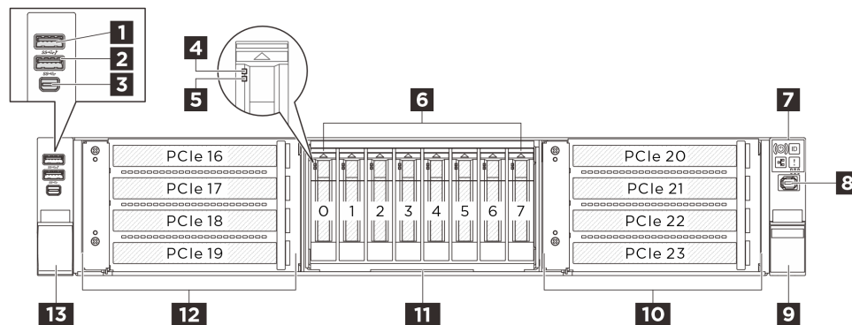
Abbildung 2. Vorderansicht der 2,5-Zoll-Laufwerkconfiguration
