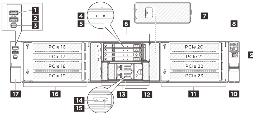
Abbildung 4. Vorderansicht der E3.S- und M.2-Laufwerkskonfiguration
