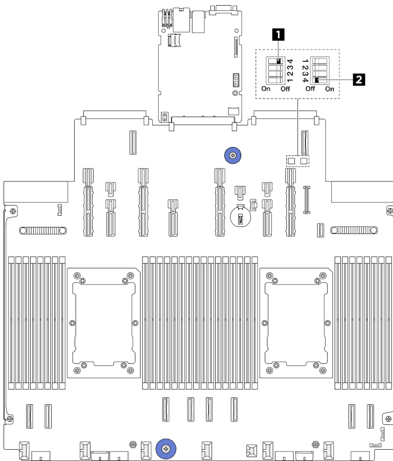
Abbildung 10. Schalter an der Systemplattenbaugruppe
