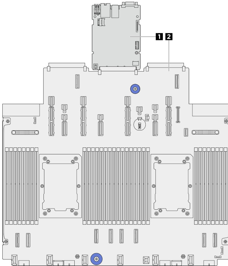
Abbildung 8. Aufbau der Systemplatinenbaugruppe
