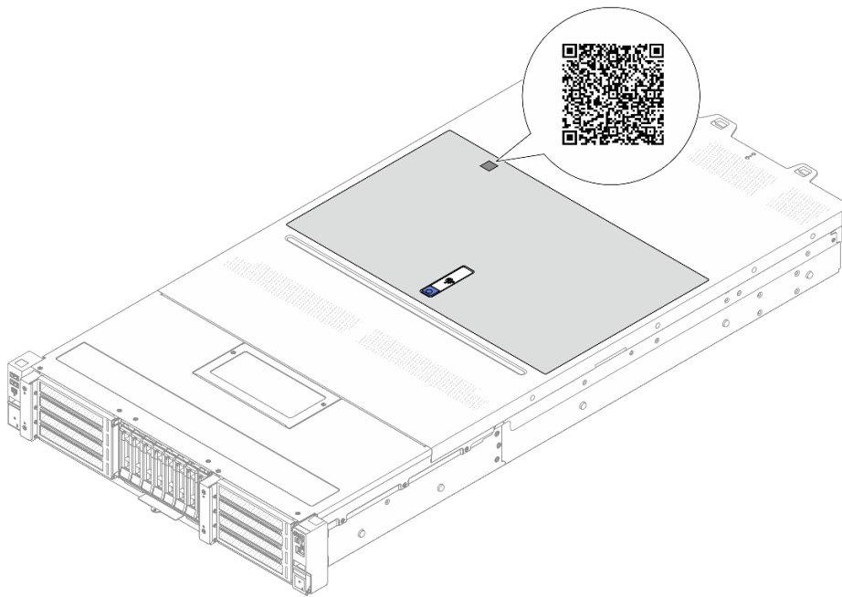
Abbildung 26. Service-Etikett und QR-Code
