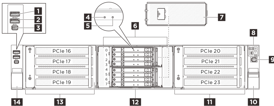
Abbildung 3. Vorderansicht der E3.S-Laufwerkskonfiguration
