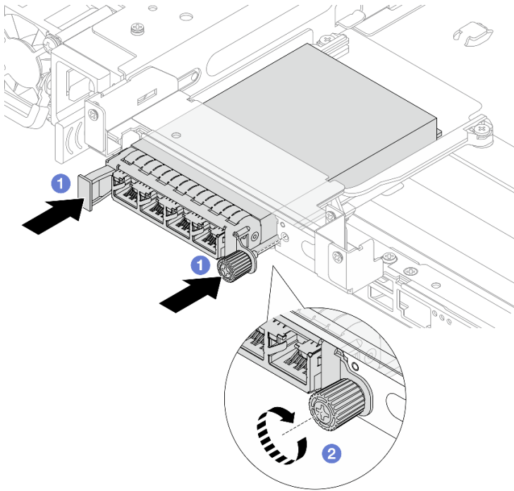
Abbildung 223. Installieren des hinteren OCP-Moduls
