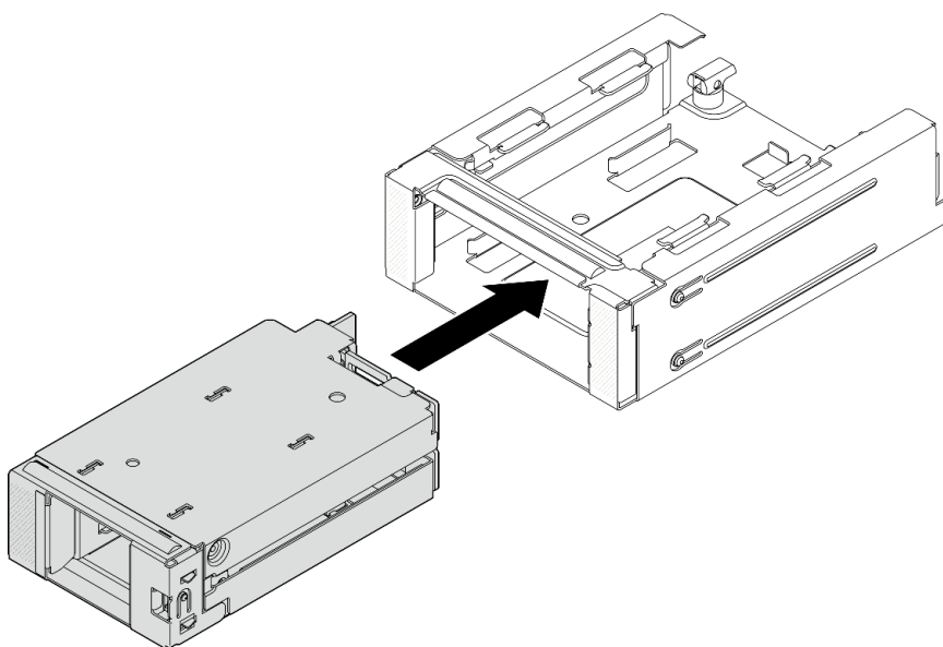
Abbildung 141. Installieren der vorderen M.2-Laufwerkhalterung im Rahmen
