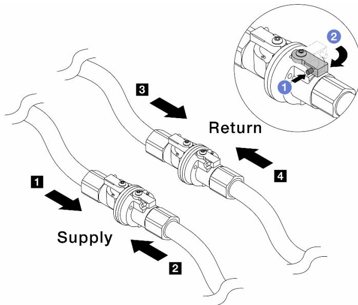
Abbildung 195. Öffnen der Kugelhähne
