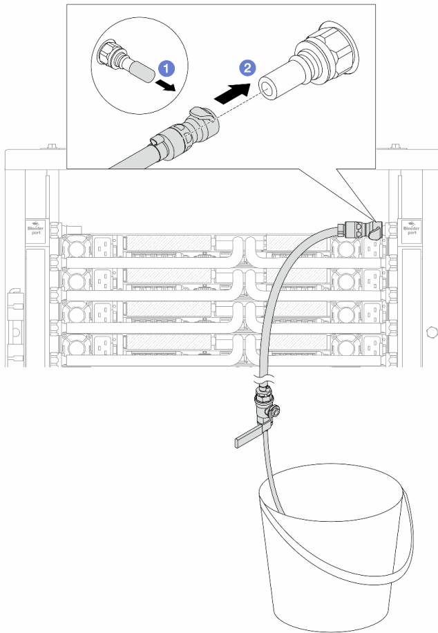
Abbildung 191. Installieren des Ablasssatzes an der Rücklaufseite
