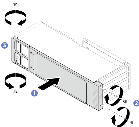
Abbildung 73. Installation der seitlichen Halterung
