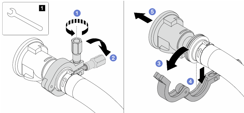
Abbildung 164. Trennen der Kugelhähne
