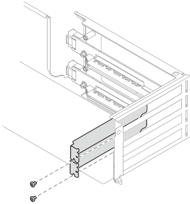
Abbildung 70. Abdeckblende für PCIe-Steckplatz
