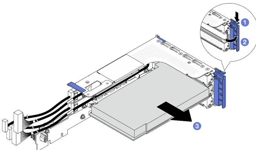
Abbildung 227. Entfernen eines PCIe-Adapters aus dem 3FH-Adapterrahmen
