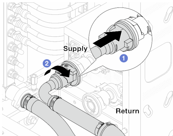
Abbildung 167. Verbinden der Kugelhähne
