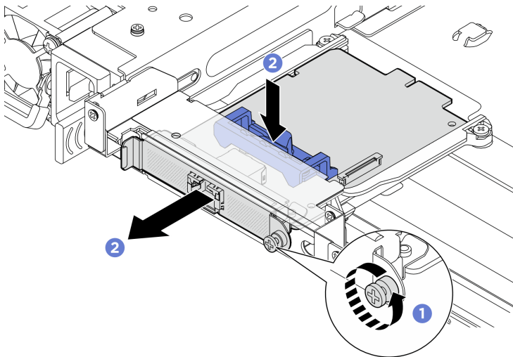
Abbildung 146. Entfernen des NIC-Verwaltungsadapters
