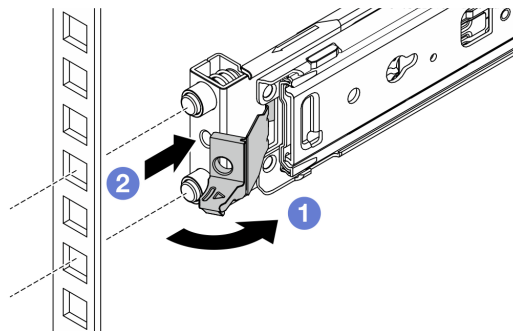
Abbildung 17. Entfernen der Schiene an der Vorderseite
