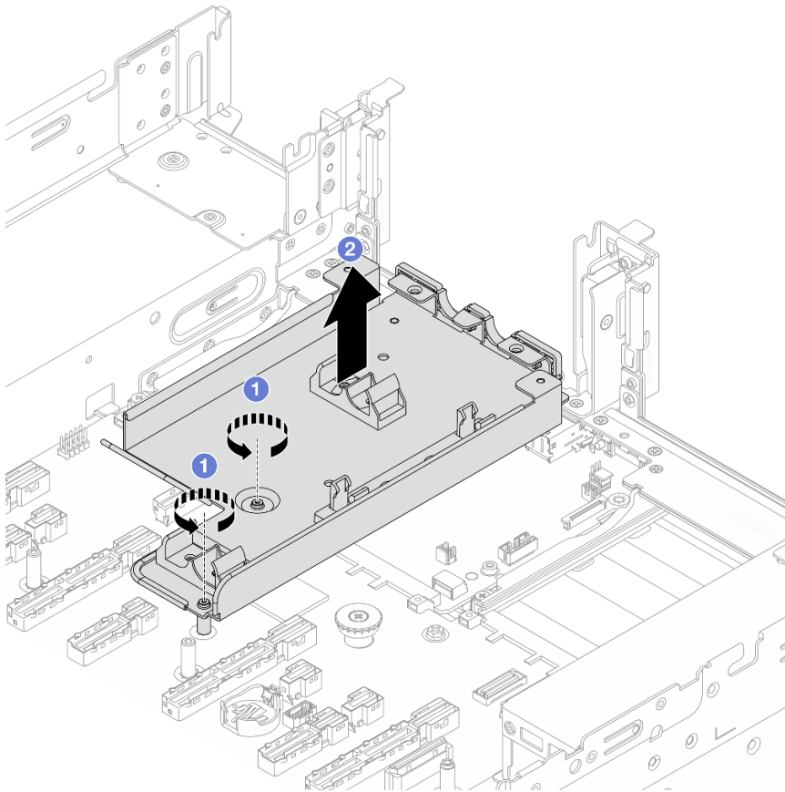
Abbildung 107. Entfernen der Schlauchhalterung
