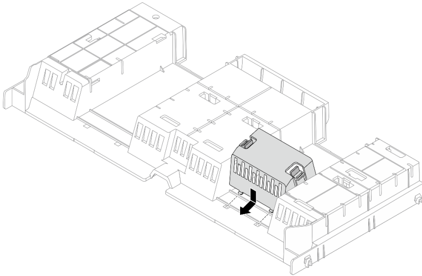
Abbildung 43. Installieren der Abdeckblenden der Luftführung
