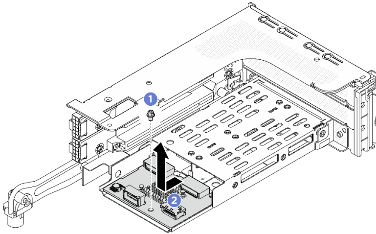
Abbildung 144. Entfernen der M.2-Rückwandplatine vom 3FH-M.2-Adapterrahmen
