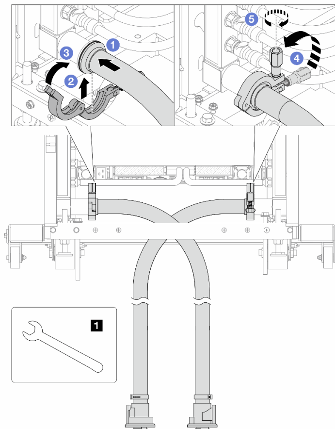
Abbildung 187. Anbringen des Schlauchsatzes
