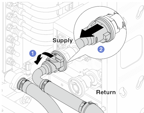
Abbildung 156. Entfernen des Verbindungssatzes
