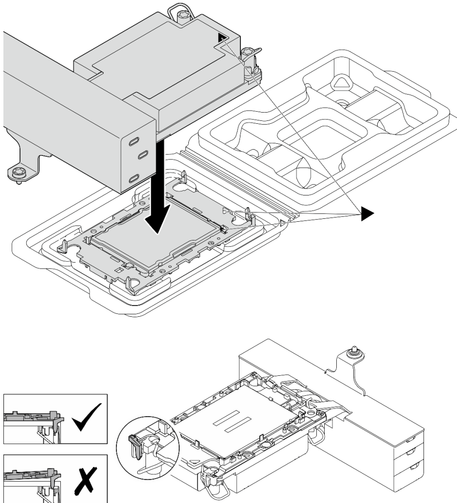
Abbildung 209. Zusammenbauen der PHM mit Prozessor im Versandeinbaurahmen
