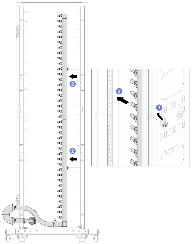
Abbildung 157. Entfernen der Leitung
