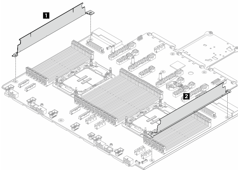
Abbildung 279. Entfernen der Kabelwände
