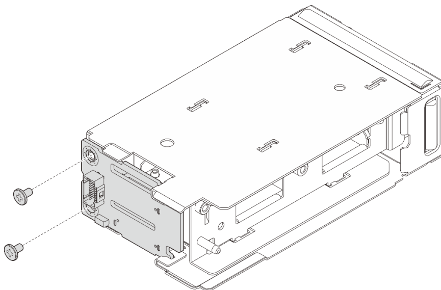
Abbildung 135. Entfernen der vorderen M.2-Boot-Rückwandplatine
