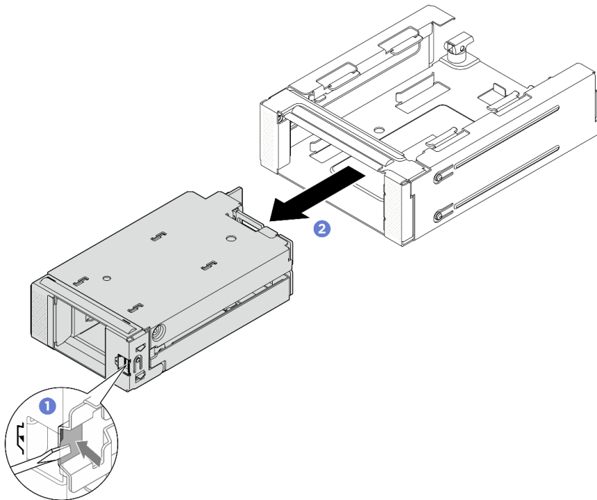
Abbildung 133. Entfernen der vorderen M.2-Laufwerkhalterung aus dem Rahmen
