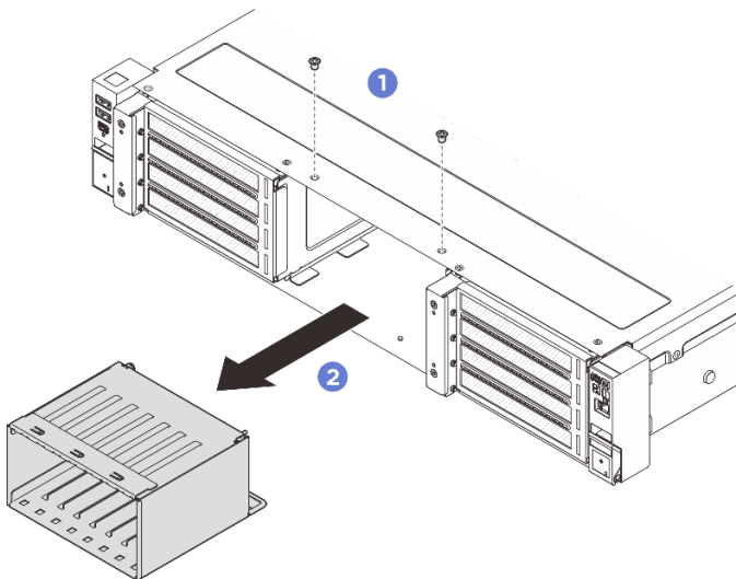
Abbildung 37. Entfernen der 2,5-Zoll-Laufwerkhalterung
