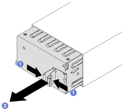
Abbildung 86. Entfernen der Abdeckblende für die Netzteilereinheit
