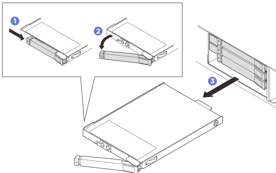
Abbildung 52. Entfernen eines E3.S-Hot-Swap-Laufwerks
