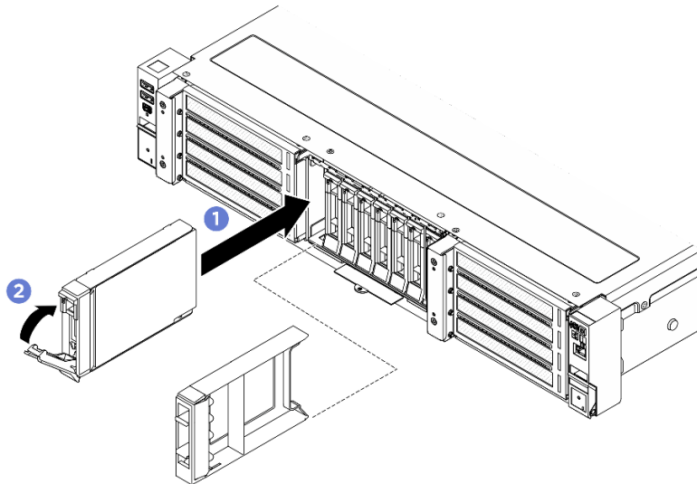
Abbildung 34. Installieren eines 2,5-Zoll-Hot-Swap-Laufwerks
