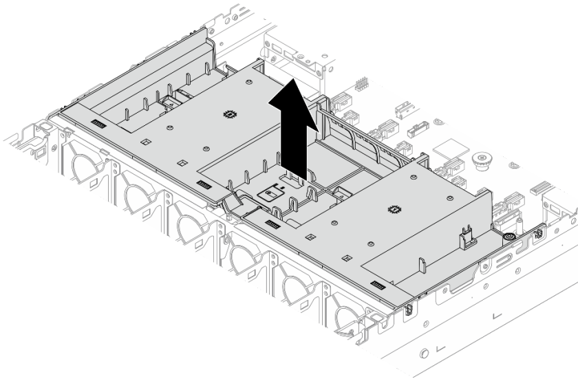
Abbildung 41. Luftführung entfernen
