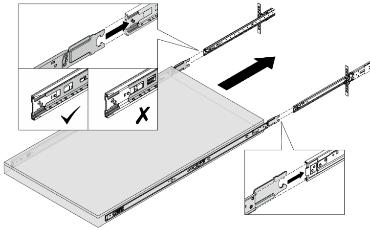
Abbildung 28. Verriegeln der Schienen
