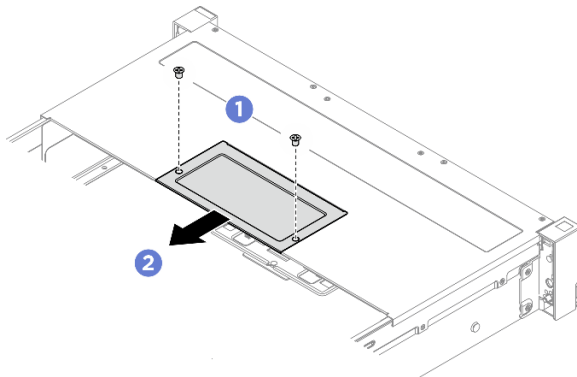
Abbildung 59. Entfernen der Abdeckplatte
