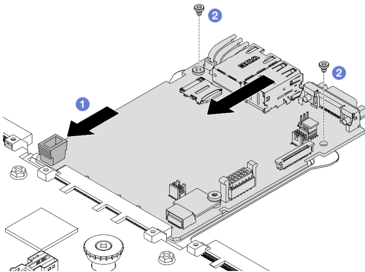
Abbildung 247. Installieren der System-E/A-Platine auf der Prozessorplatine
