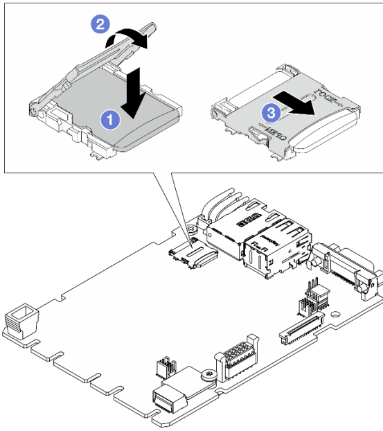
Abbildung 199. Installieren der microSD-Karte
