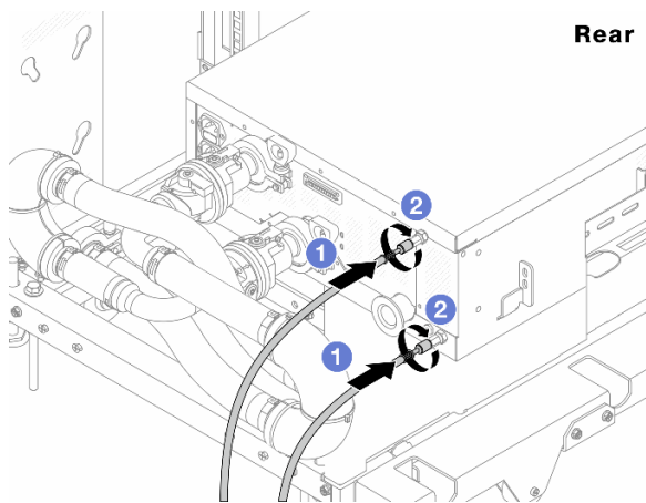
Abbildung 169. Rückseite des Kühlwasserverteilers
