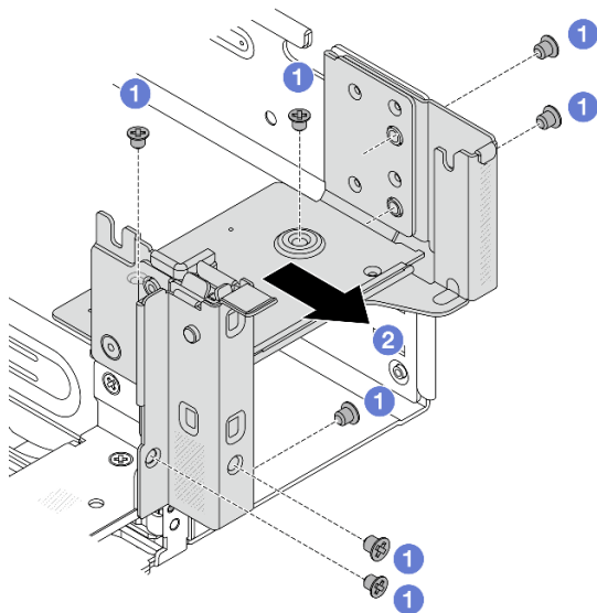
Abbildung 234. Entfernen der rechten Rückwandhalterung
