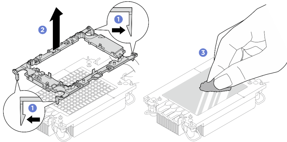
Abbildung 205. Trennen eines Prozessorträgers vom Kühlkörper
