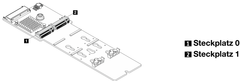
Abbildung 94. M.2-Laufwerksteckplätze
