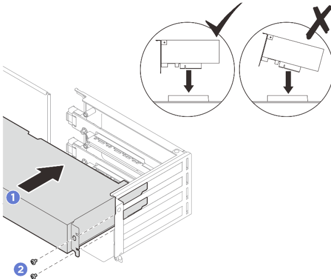
Abbildung 71. Installation des PCIe-Adapters
