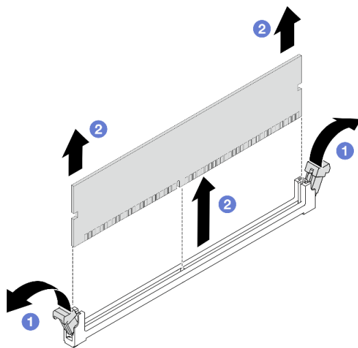
Abbildung 196. Entfernen des Speichermoduls
