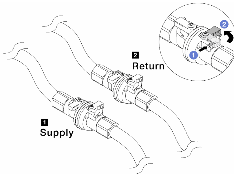
Abbildung 177. Schließen der Kugelhähne
