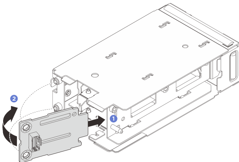
Abbildung 138. M.2-Boot-Rückwandplatine installieren
