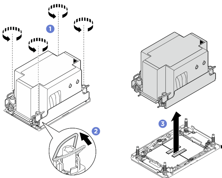
Abbildung 201. Entfernen eines 2U-Standard-PHM
