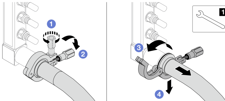
Abbildung 184. Trennen der Leitung vom Schlauchsatz
