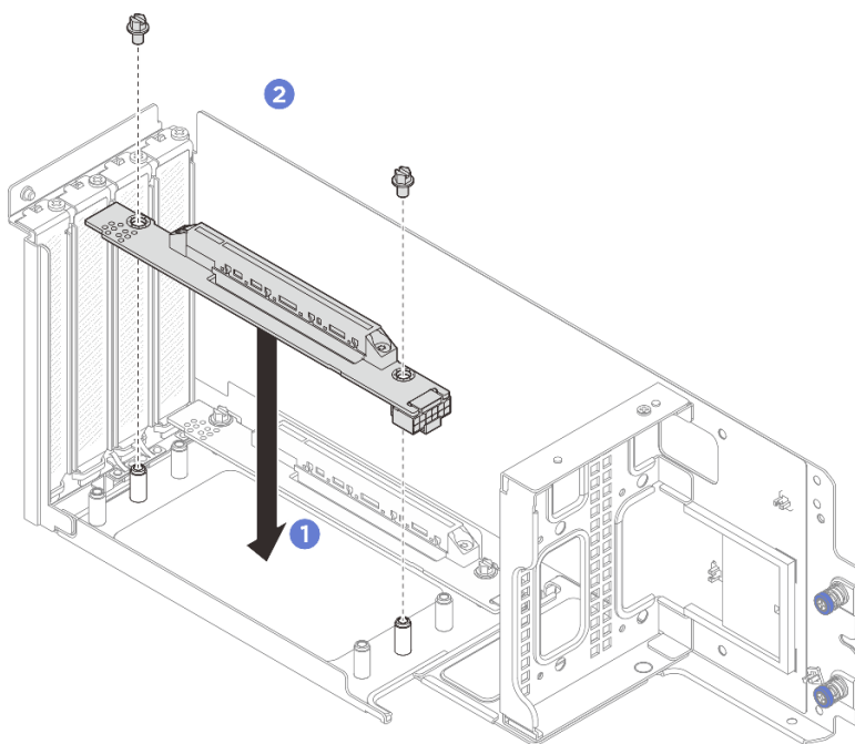
Abbildung 77. Installation einer Adapterkarte
