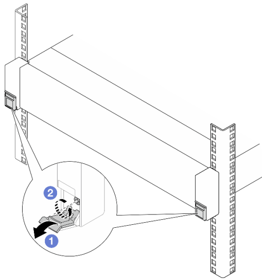
Abbildung 21. Trennen des Servers aus dem Rack
