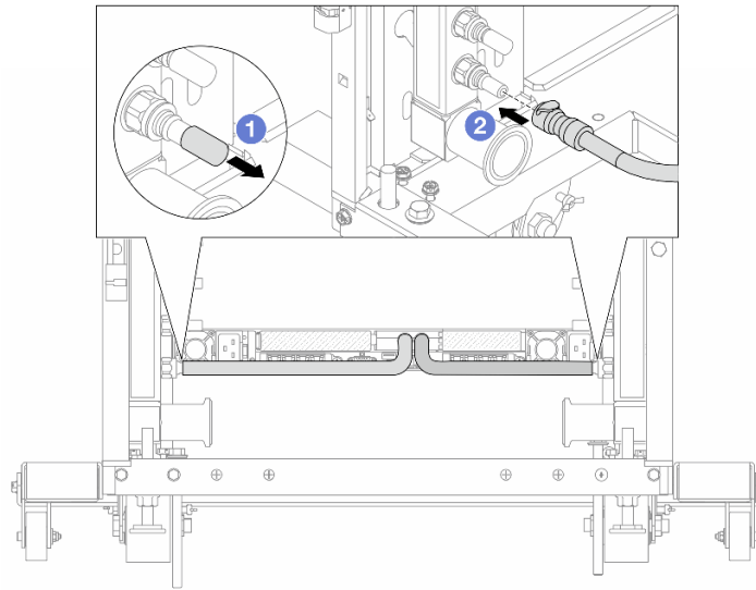
Abbildung 186. Anbringen der Schnellanschlüsse
