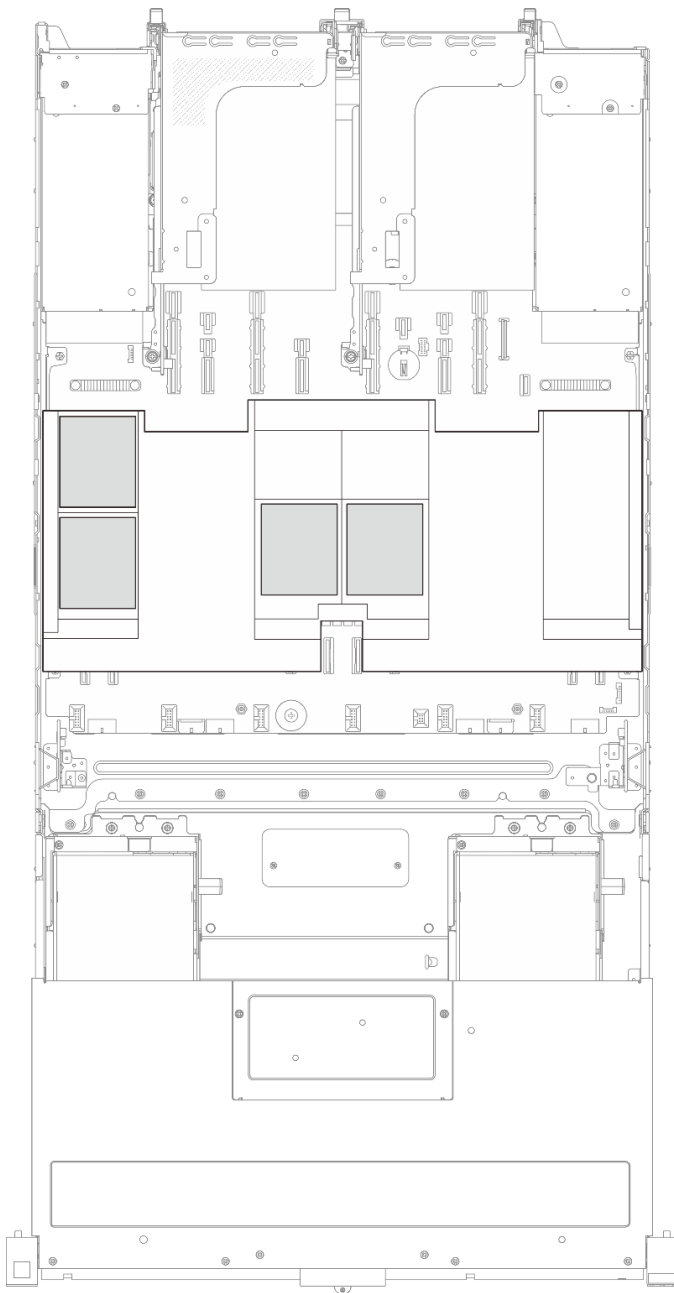
Abbildung 219. Position des RAID-Flashstromversorgungsmoduls an der Luftführung
