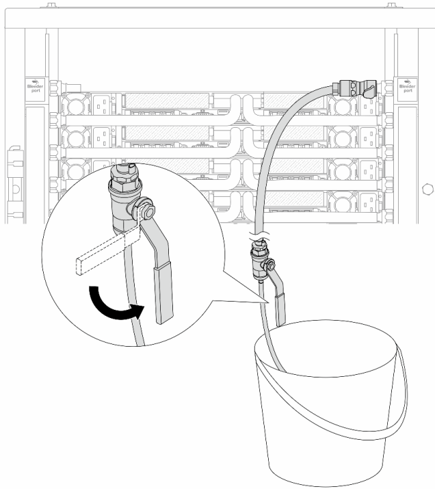
Abbildung 175. Öffnen des Ablassventils an der Rücklaufseite
