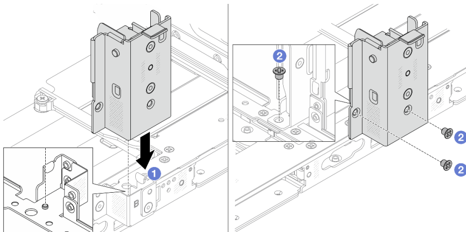
Abbildung 236. Installieren der mittleren Rückwandhalterung
