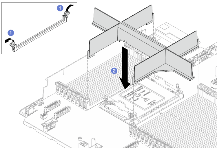
Abbildung 203. Installieren einer PHM-Abdeckblende
