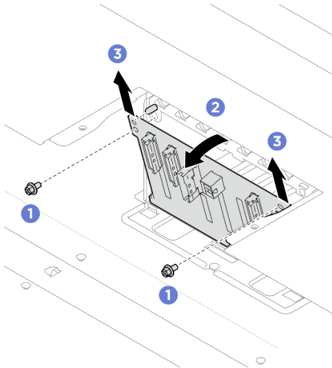
Abbildung 36. Entfernen der Rückwandplatine für 2,5-Zoll-Laufwerke
