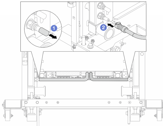
Abbildung 170. Anbringen der Schnellanschlüsse
