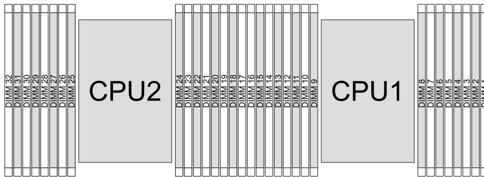
Abbildung 15. Speichermodul-Steckplätze auf der Prozessorplatine
