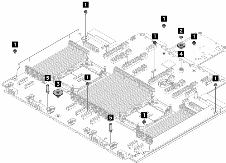
Abbildung 278. Zerlegen der Systemplattenbaugruppe
