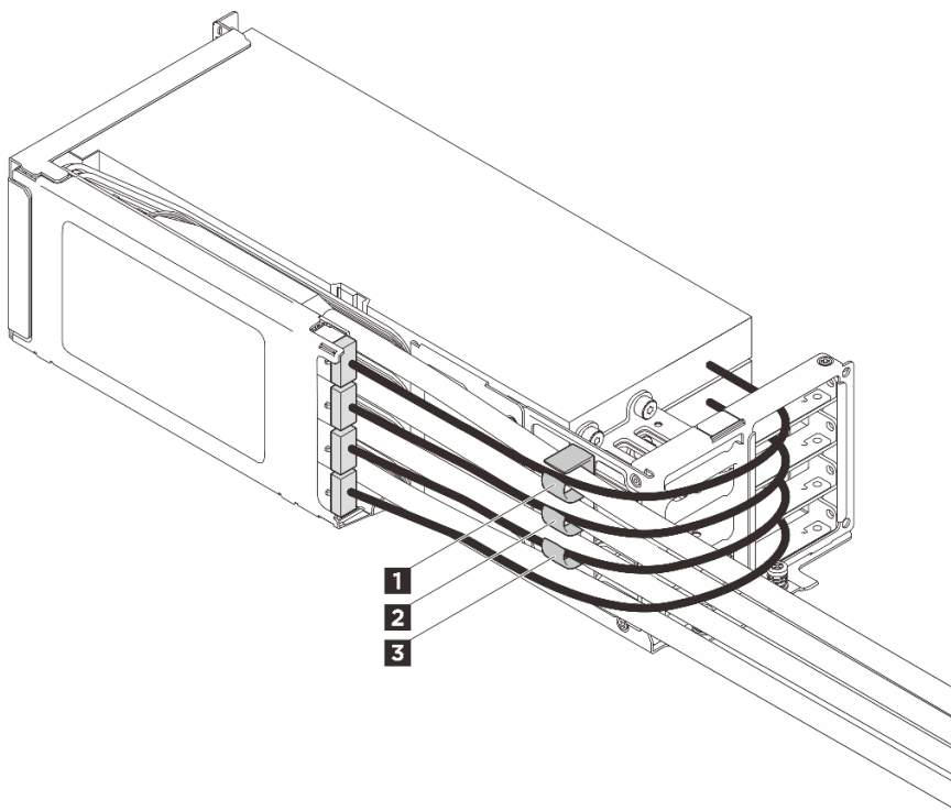
Abbildung 75. Kabelklemmen der Adapterkartenbaugruppe an der Vorderseite
