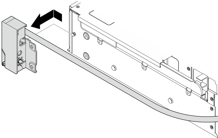
Abbildung 215. Entfernen der Rack-Verriegelung
