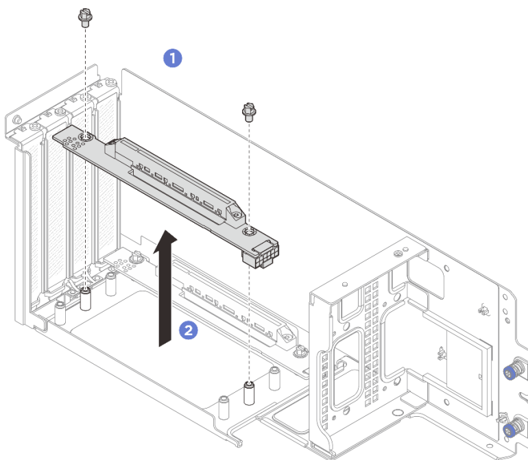
Abbildung 76. Ausbau der Adapterkarte
