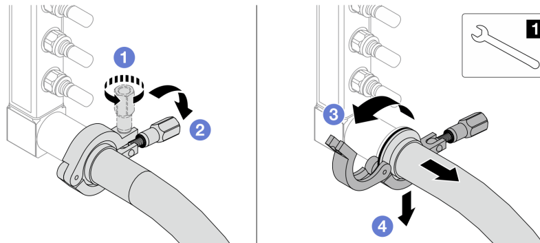
Abbildung 162. Trennen der Leitung vom Verbindungssatz
