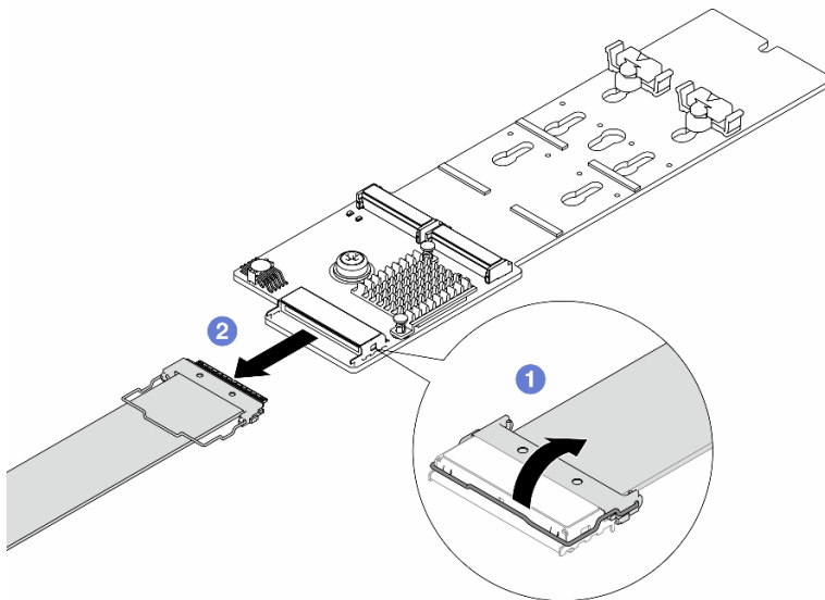
Abbildung 96. Abziehen des M.2-Kabels
