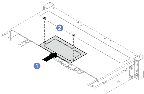
Abbildung 40. Installieren der Abdeckplatte
