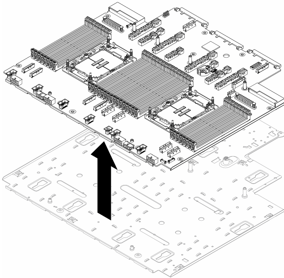
Abbildung 280. Entfernen der Prozessorplatine
