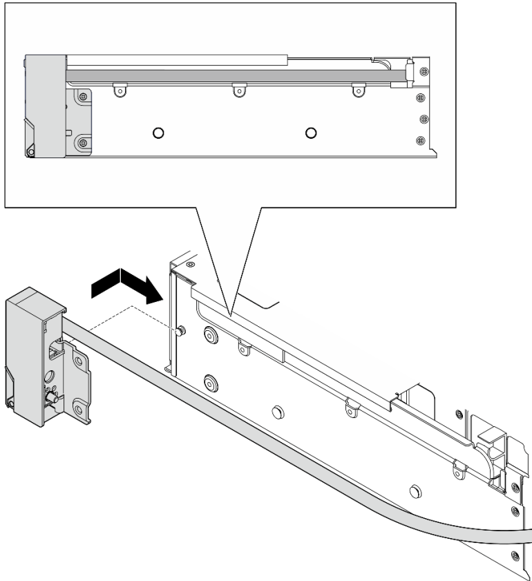
Abbildung 216. Installieren der Rack-Verriegelung
