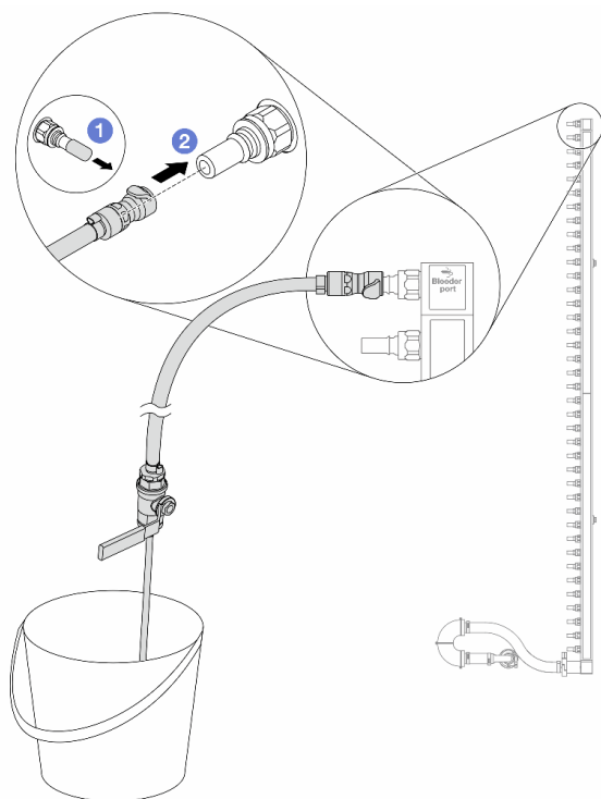
Abbildung 160. Installieren des Ablasssatzes an der Rücklaufseite
