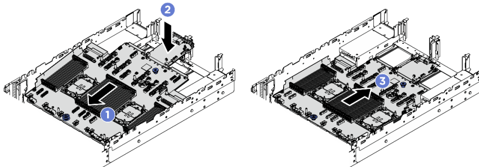
Abbildung 248. Installieren der Systemplatinenbaugruppe
