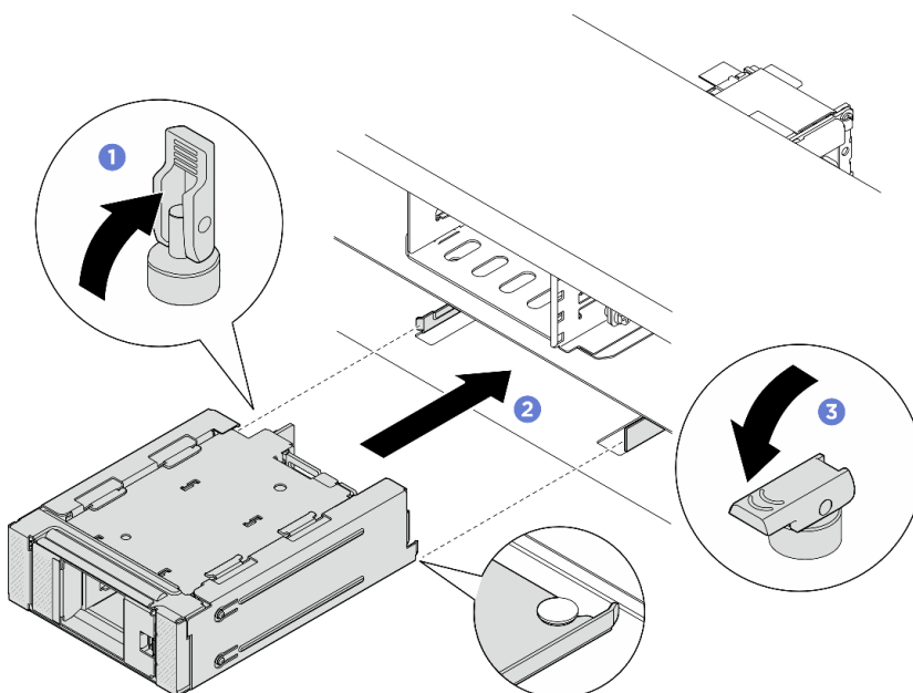
Abbildung 142. Installieren der vorderen M.2-Laufwerkhalterung mit Rahmen
