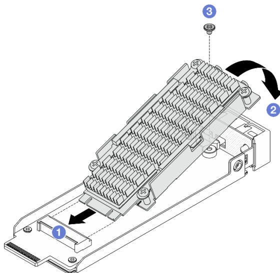
Abbildung 130. Installieren des M.2-Laufwerks mit Kühlkörper
