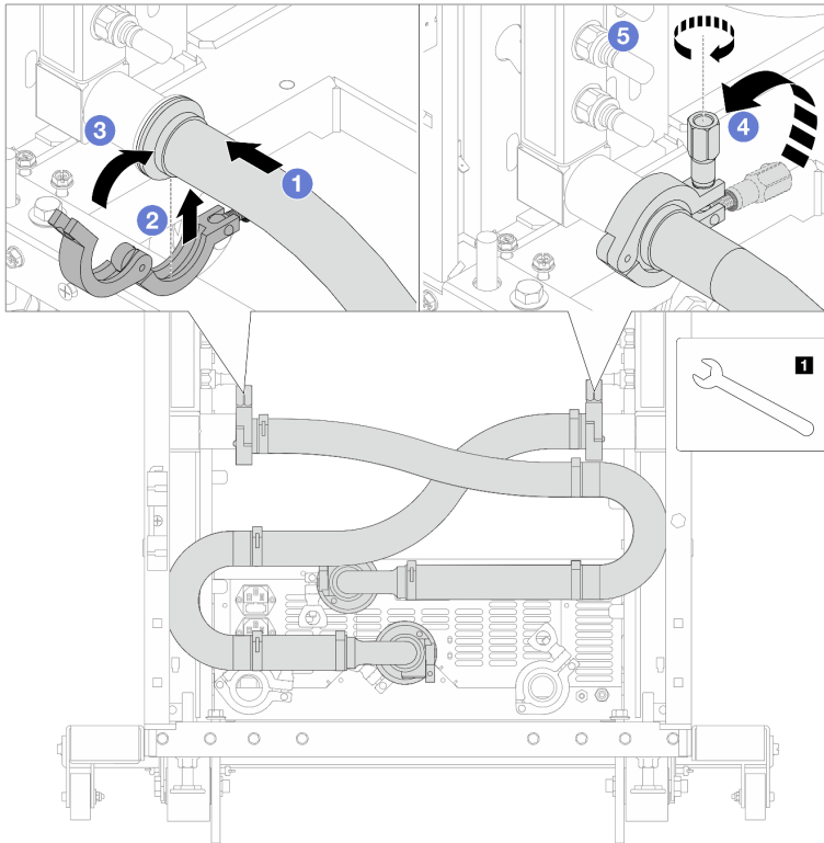
Abbildung 166. Anbringen des Verbindungssatzes
