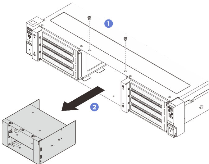
Abbildung 62. Entfernen der E3.S-Laufwerkhalterung
