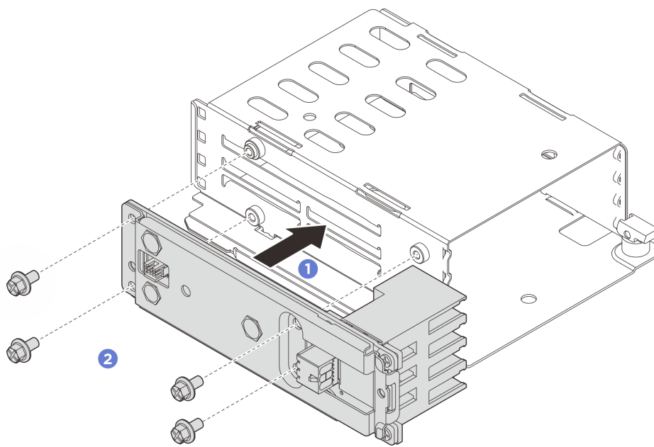
Abbildung 64. Installieren der Rückwandplatinenbaugruppe
