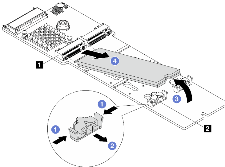
Abbildung 92. M.2-Laufwerk entfernen
