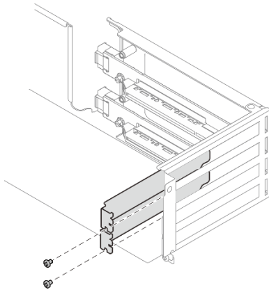
Abbildung 69. Abdeckblende für PCIe-Steckplatz
