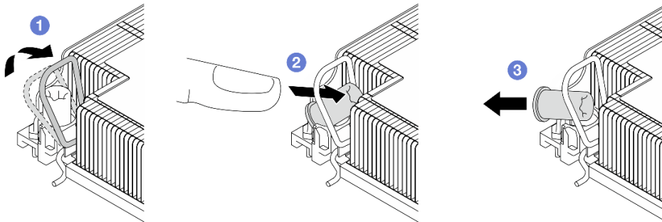
Abbildung 79. Entfernen einer T30-Torx-Mutter vom Kühlkörper
