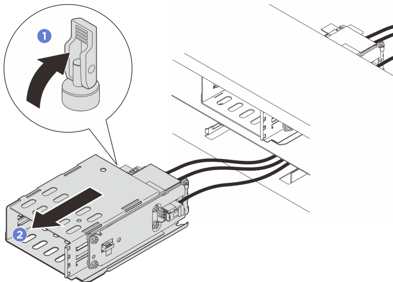
Abbildung 60. Entfernen der E3.S-1T-Halterung
