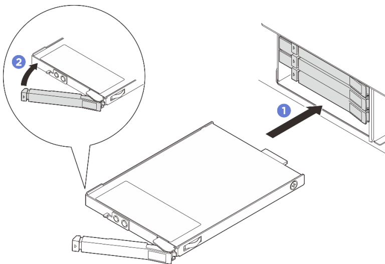
Abbildung 55. Installieren eines E3.S-Hot-Swap-Laufwerks
