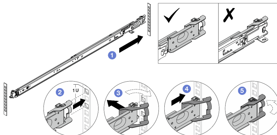
Abbildung 19. Installieren der hinteren Befestigungsstifte
