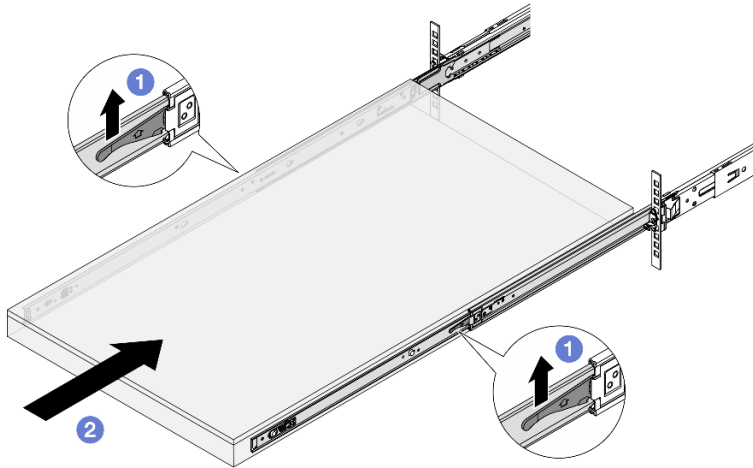
Abbildung 29. Verriegeln der Schienen und Einschieben in den Server
