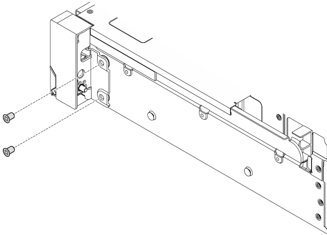
Abbildung 217. Installieren der Schrauben
