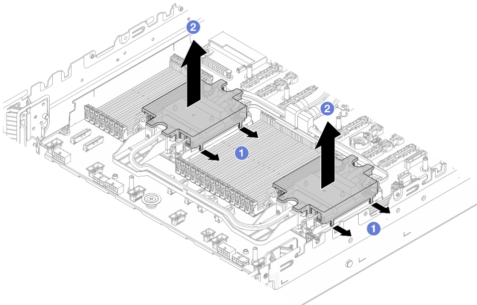
Abbildung 277. Entfernen der Kühlplattenabdeckung
