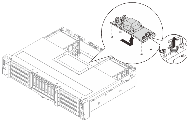
Abbildung 90. Entfernen des internen CFF-Adapters
