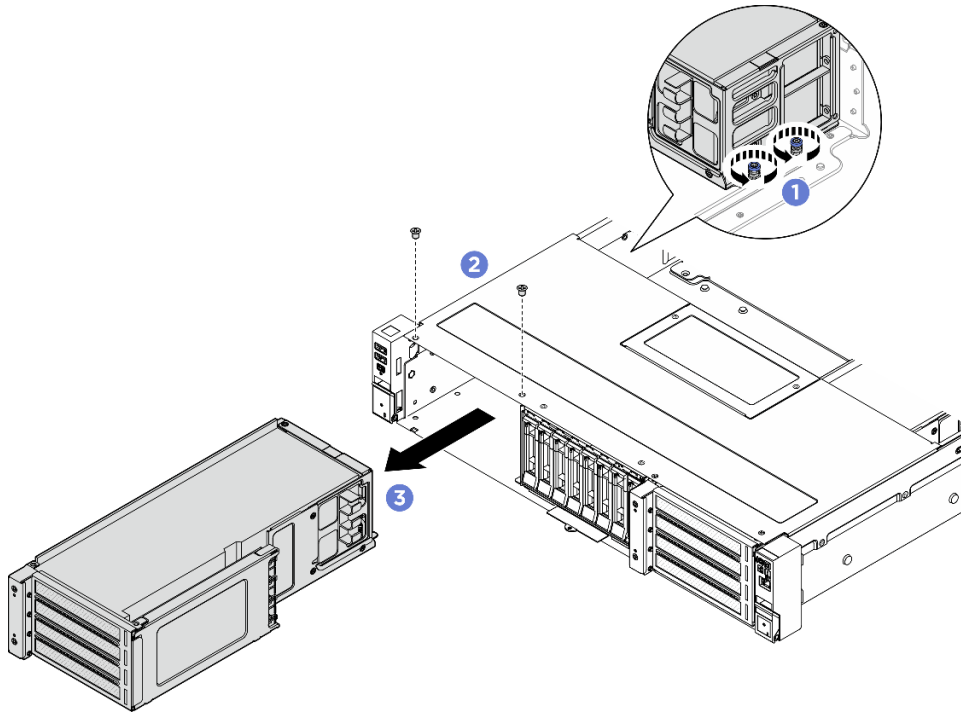
Abbildung 66. Entfernen der vorderen Adapterkartenbaugruppe
