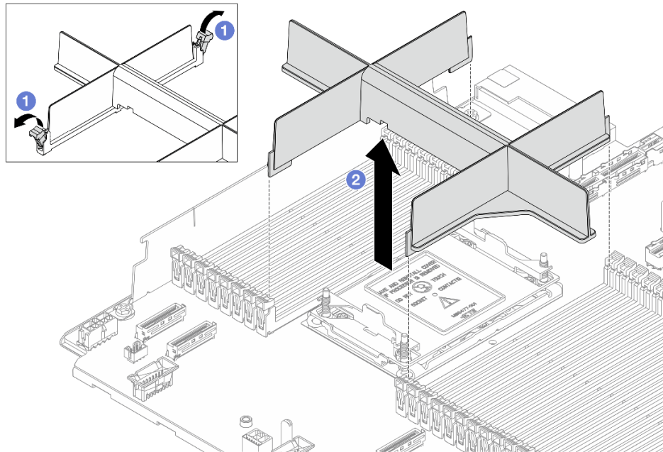
Abbildung 210. Entfernen einer PHM-Abdeckblende
