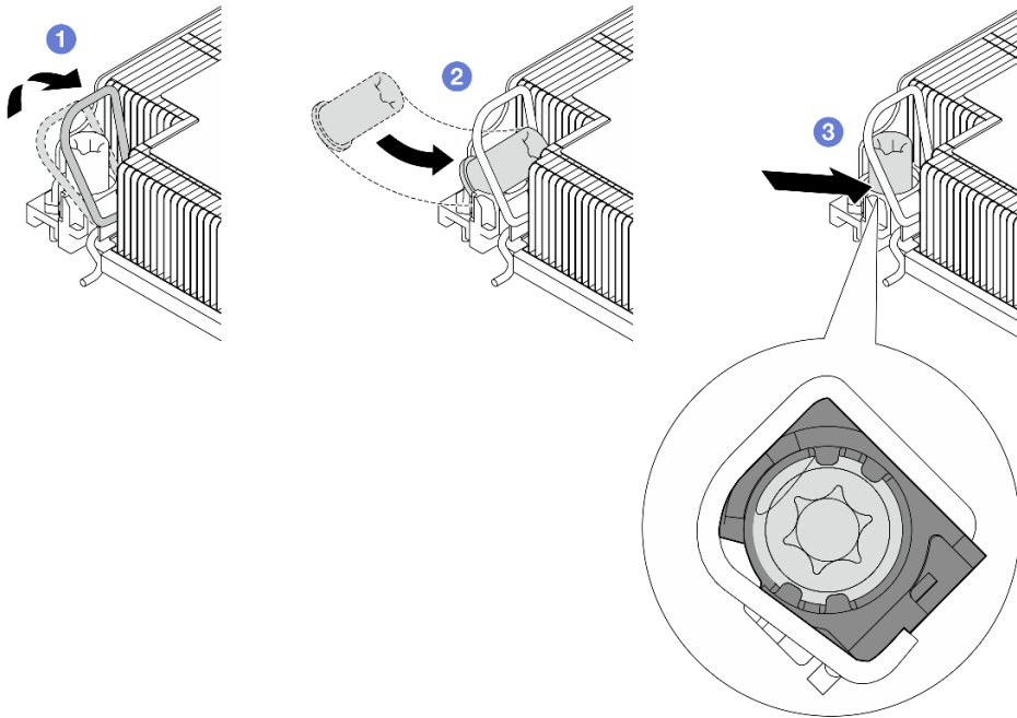
Abbildung 80. Anbringen einer T30-Torx-Mutter am Kühlkörper
