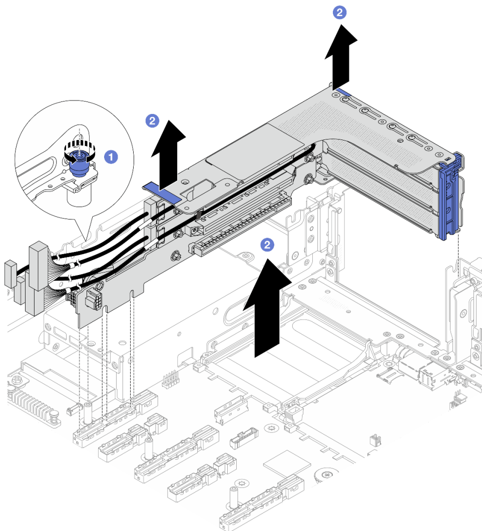
Abbildung 226. Entfernen der 3FH-Adapterkartenbaugruppe
