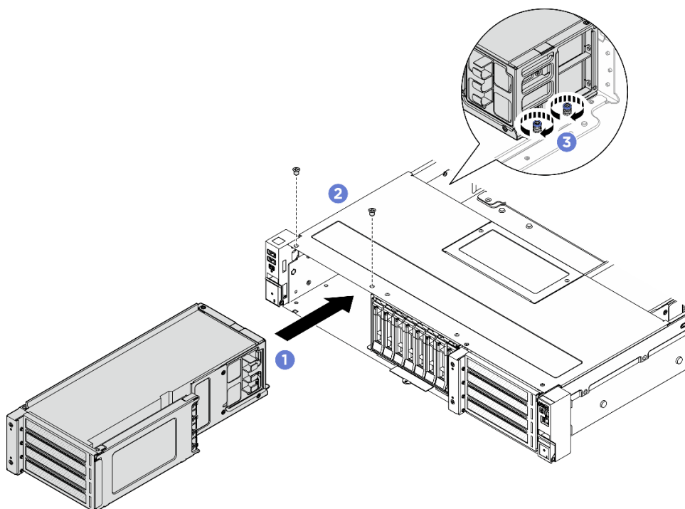
Abbildung 74. Installation der Adapterkartenbaugruppe an der Vorderseite
