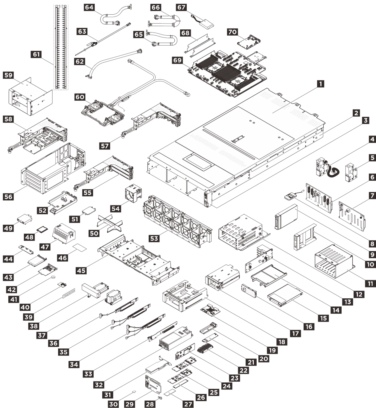
Abbildung 11. Serverkomponenten
