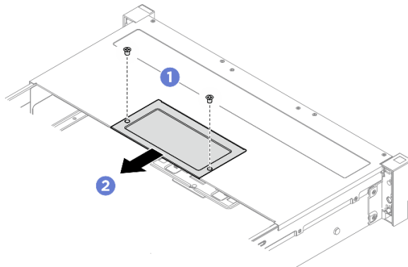
Abbildung 89. Entfernen der Abdeckplatte
