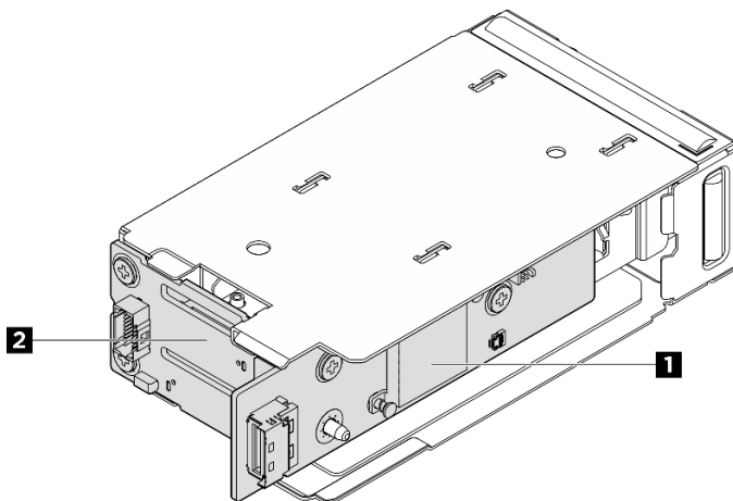
Abbildung 131. Vordere Rückwandplatinen für M.2-Laufwerke
