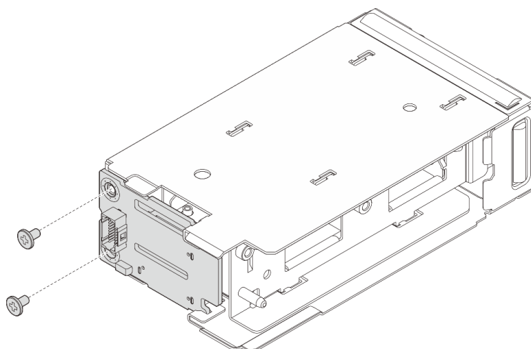
Abbildung 139. M.2-Boot-Rückwandplatte installieren
