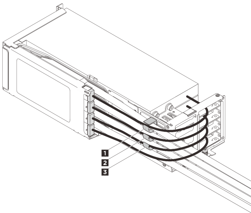
Abbildung 78. Kabelklemmen der Adapterkartenbaugruppe an der Vorderseite
