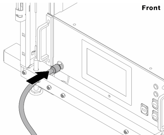
Abbildung 168. Vorderseite des Kühlwasserverteilers
