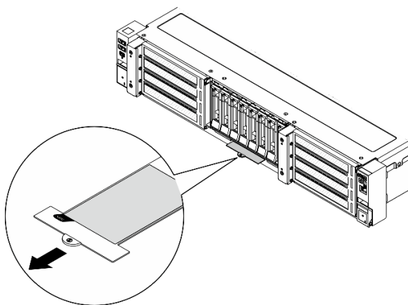
Abbildung 13. Position des Lenovo XClarity Controller-Netzwerkzugriffsetiketts auf der herausziehbaren Informationskarte
