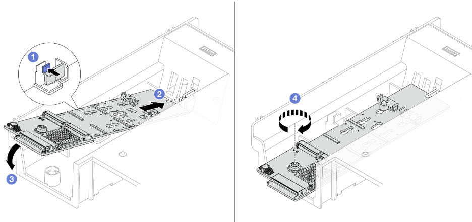
Abbildung 98. Installieren der M.2-Rückwandplatine an der Luftführung
