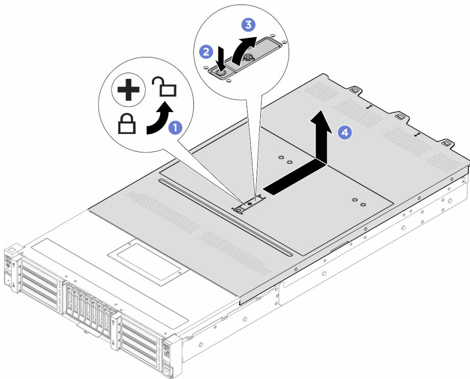
Abbildung 257. Entfernen der oberen Abdeckung
