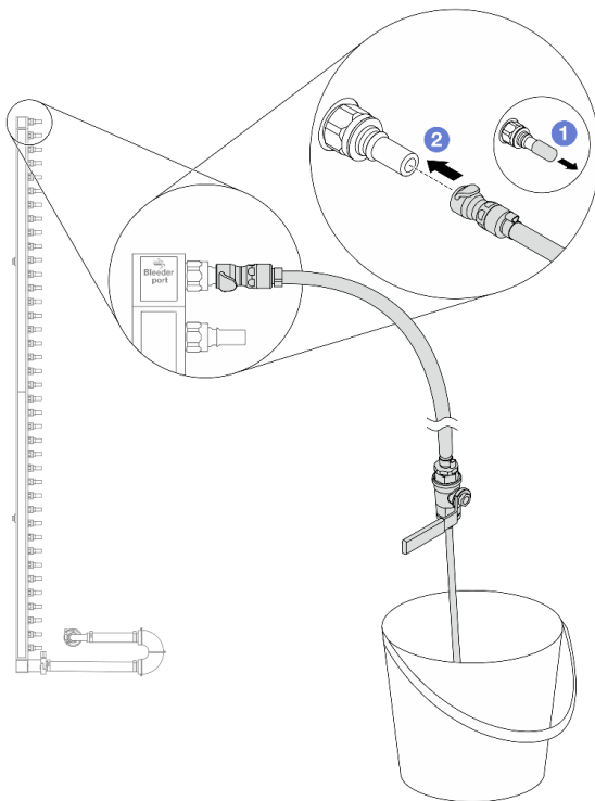
Abbildung 158. Installieren des Ablasssatzes an der Zulaufseite
