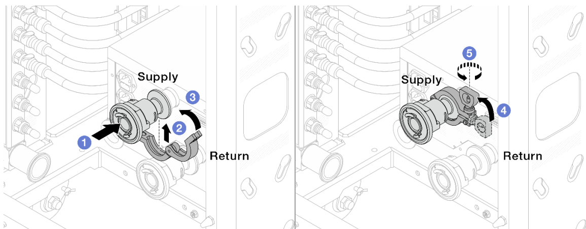
Abbildung 165. Installieren der Kugelhähne
