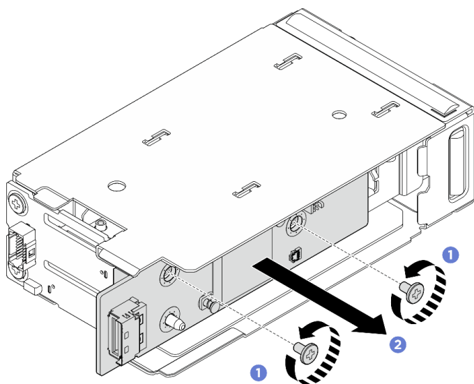
Abbildung 134. Entfernen der vorderen M.2-Controllerplatine
