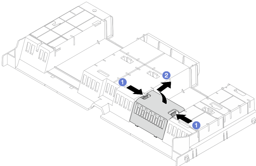
Abbildung 42. Entfernen der Abdeckblende der Luftführung
