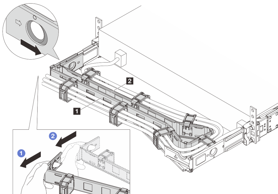
Abbildung 82. Entfernen der linken Seite
