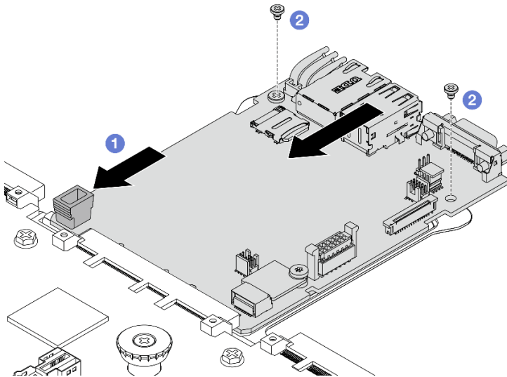
Abbildung 251. Installieren der System-E/A-Platine auf der Prozessorplatine
