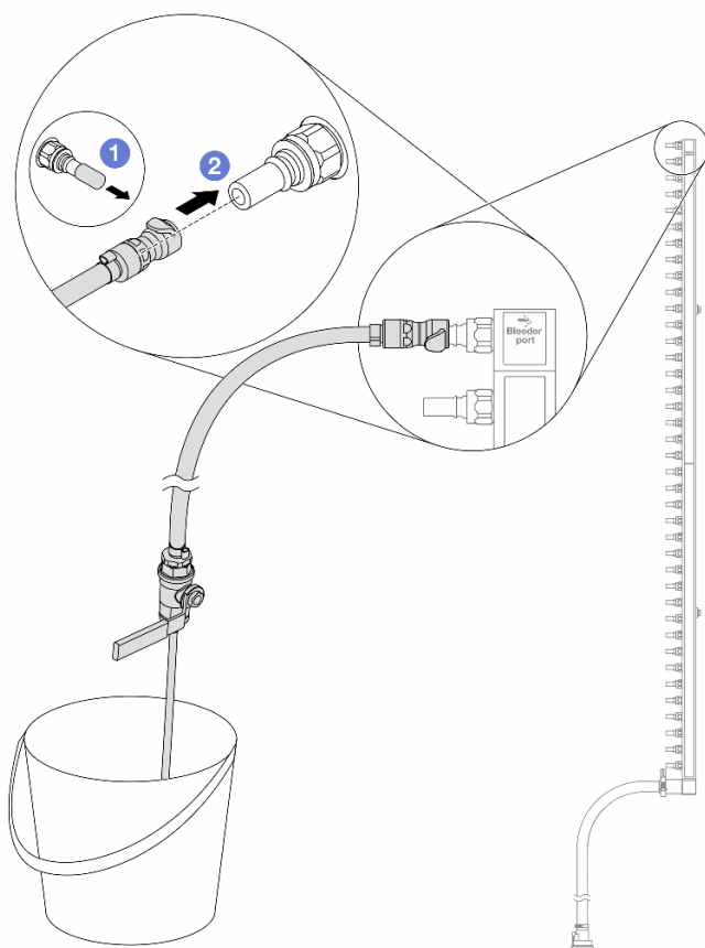
Abbildung 182. Installieren des Ablasssatzes an der Rücklaufseite
