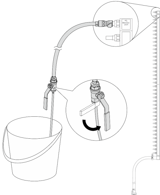
Abbildung 183. Öffnen des Ablassventils
