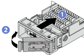
Abbildung 122. Installieren einer M.2-Laufwerkbaugruppe
