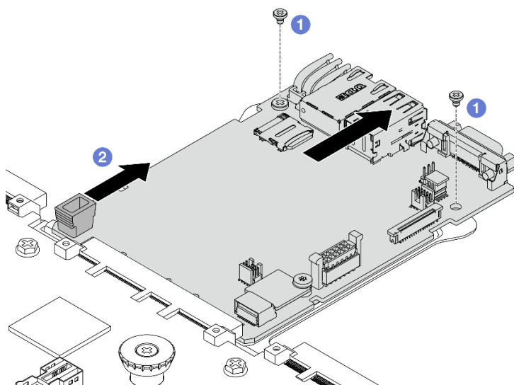
Abbildung 246. Trennen der System-E/A-Platine von der Prozessorplatine
