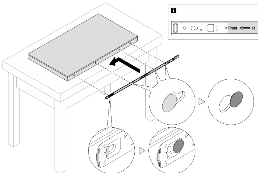
Abbildung 26. Installieren der inneren Schienen
