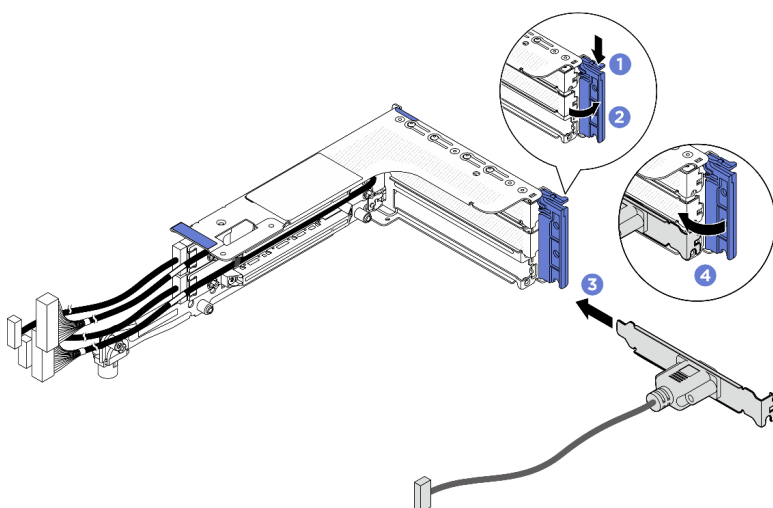
Abbildung 242. Serielles Anschlussmodul installieren
