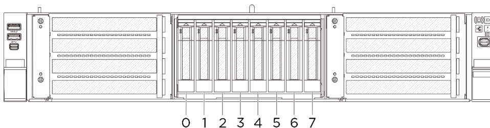
Abbildung 33. Nummerierung der 2,5-Zoll-Laufwerkpositionen
