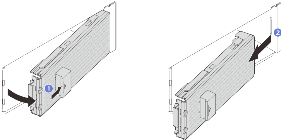
Abbildung 53. Entfernen der E3.S-Blende
