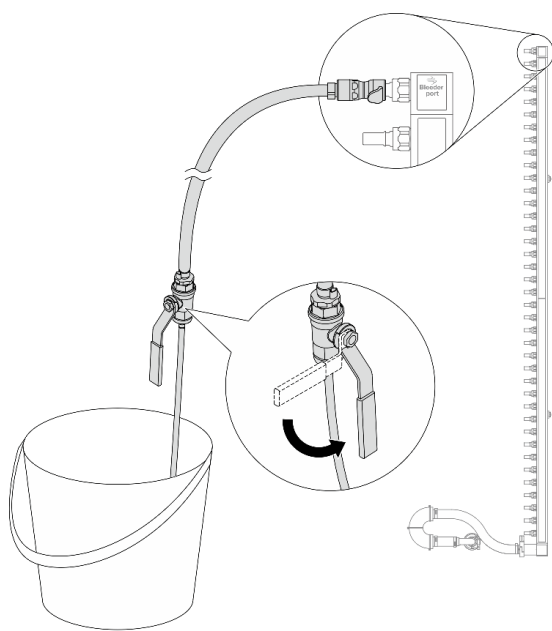
Abbildung 161. Öffnen des Ablassventils
