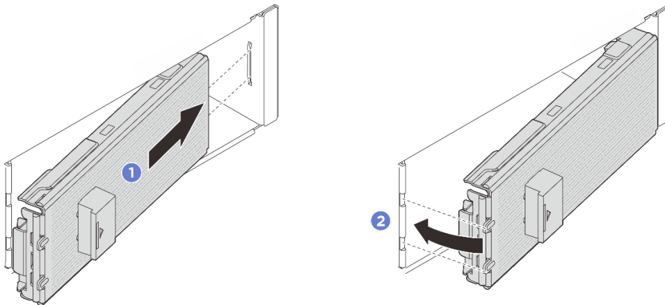
Abbildung 58. Installieren der E3.S-Blende
