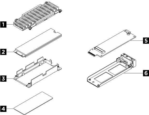
Abbildung 118. Teile einer Hot-Swap-M.2-Laufwerkbaugruppe
