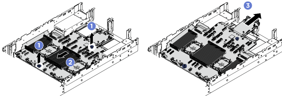
Abbildung 245. Entfernen der Systemplatinenbaugruppe
