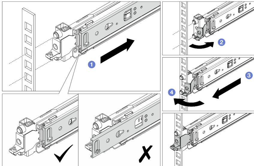
Abbildung 20. Installieren der vorderen Befestigungsstifte
