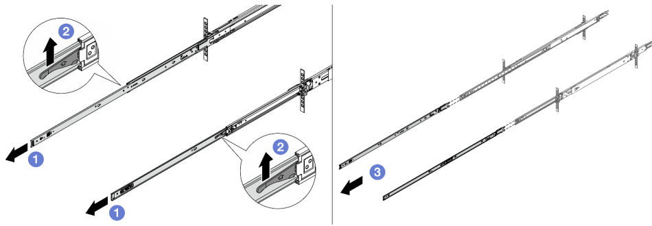
Abbildung 25. Herausziehen der Schienen
