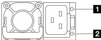
Abbildung 271. Anzeigen an einer CRPS Premium Netzteileneinheit
