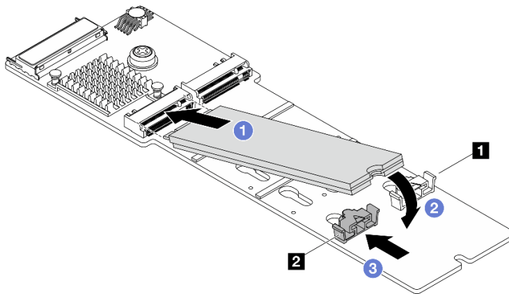
Abbildung 95. M.2-Laufwerk installieren
