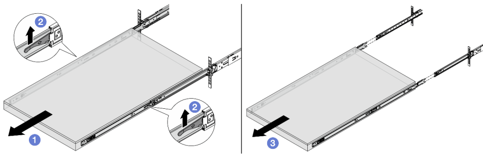
Abbildung 23. Herausziehen des Servers
