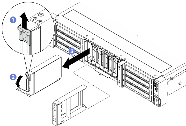
Abbildung 32. Entfernen eines 2,5-Zoll-Hot-Swap-Laufwerks
