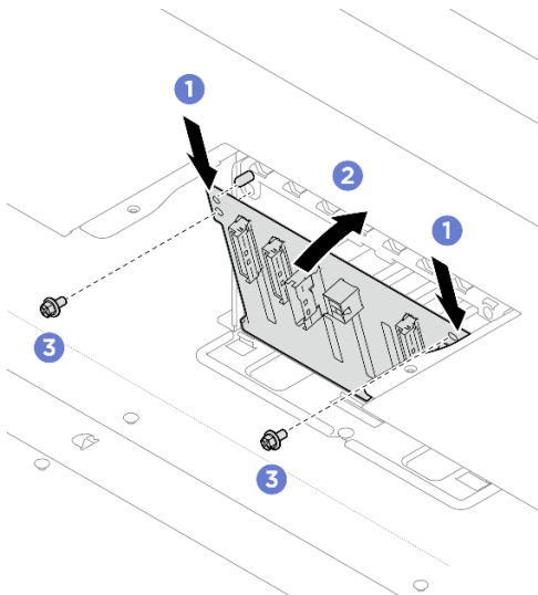
Abbildung 39. Installieren der Rückwandplatine für 2,5-Zoll-Laufwerke
