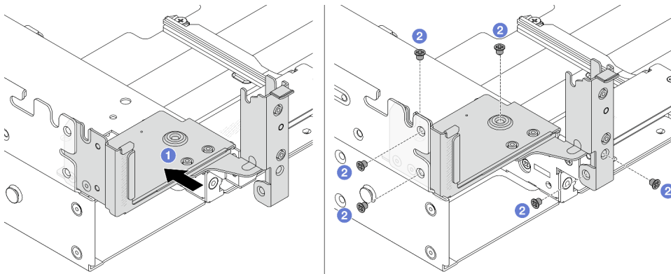
Abbildung 235. Installieren der linken Rückwandhalterung
