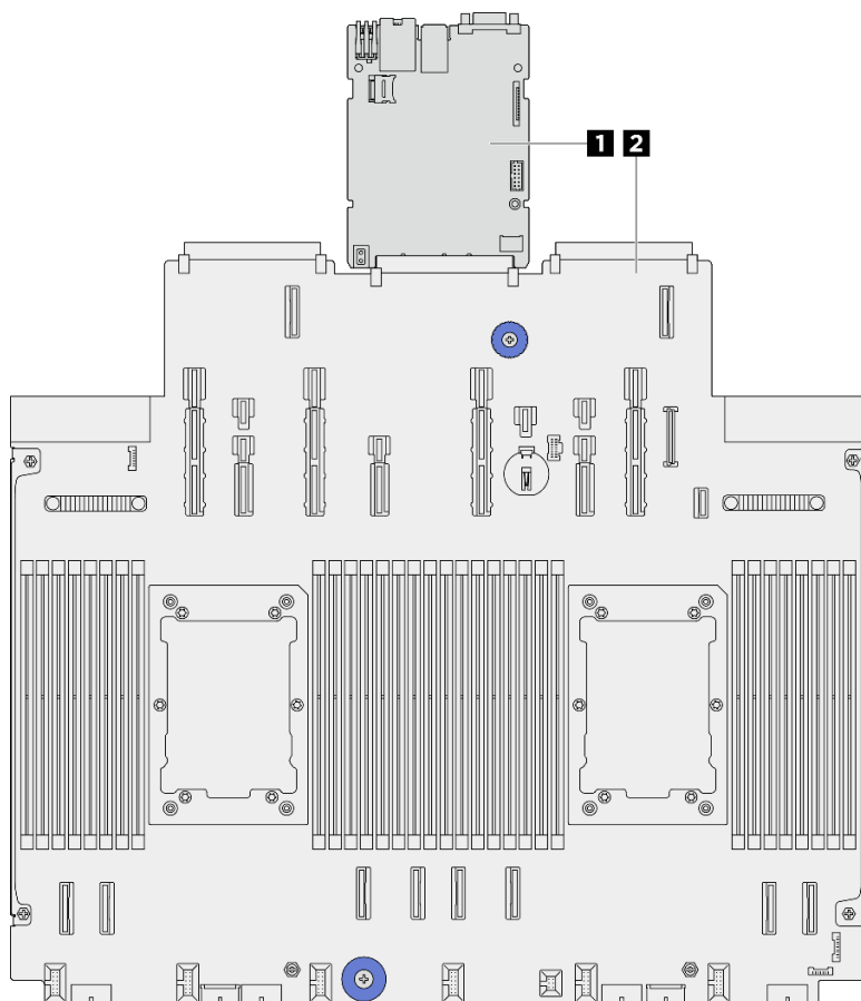
Abbildung 244. Aufbau der Systemplatinenbaugruppe
