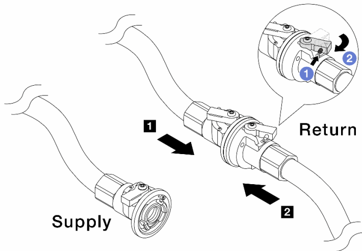
Abbildung 189. Versorgungsschlauch zu Rücklaufleitung
