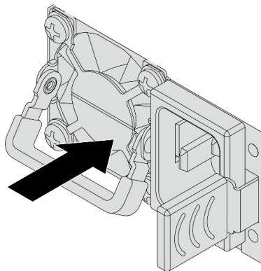
Abbildung 87. Installieren der Hot-Swap-Netzteilereinheit
