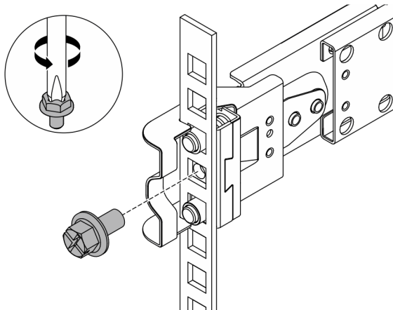
Abbildung 16. Entfernen der M6-Schrauben
