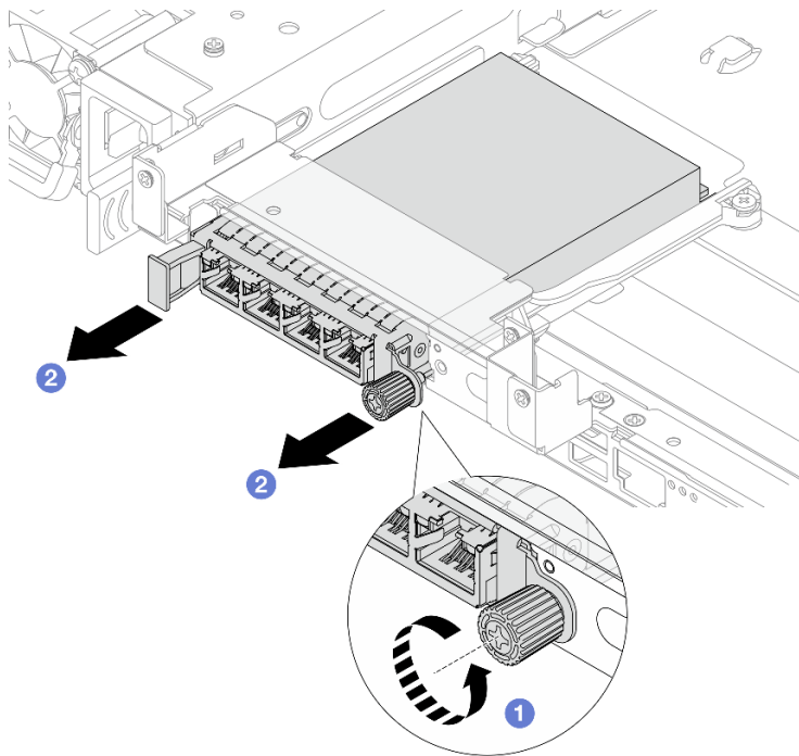
Abbildung 222. Herausnehmen des hinteren OCP-Moduls
