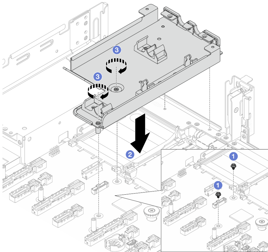
Abbildung 108. Installieren der Schlauchhalterung
