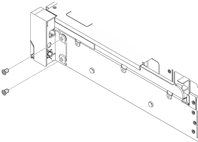
Abbildung 214. Entfernen der Schrauben
