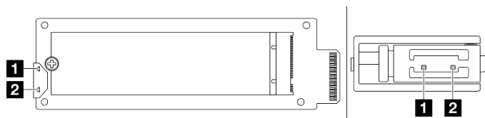
Abbildung 269. Anzeigen am M.2-Interposer
