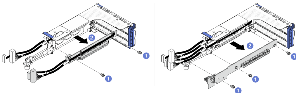
Abbildung 228. Entfernen der Adapterkarten aus dem Adapterrahmen
