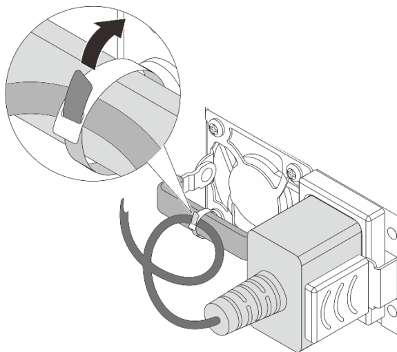
Abbildung 88. Verlegen und Festbinden des Netzkabels
