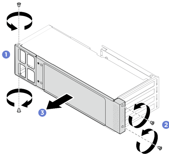
Abbildung 67. Entfernen der seitlichen Halterung
