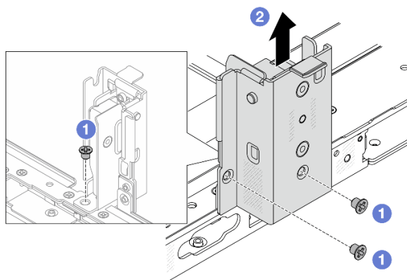
Abbildung 232. Entfernen der linken Rückwandhalterung
