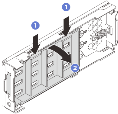
Abbildung 57. Entfernen der inneren Platte
