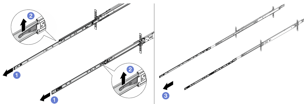
그림 7. 내부 레일 제거
