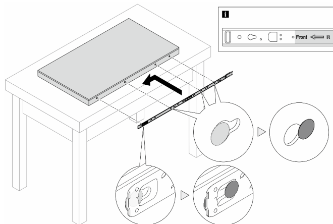
그림 8. 서버에 내부 레일 설치
