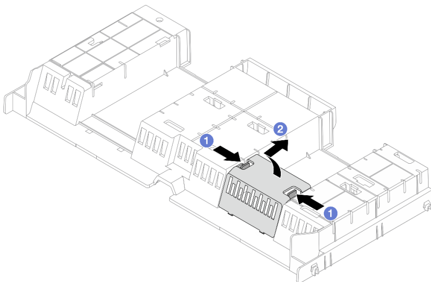
Figura 28. Removendo o preenchimento do defletor de ar
