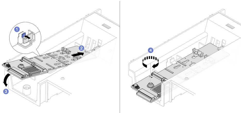
Figura 84. Instalando o backplane M.2 no defletor de ar
