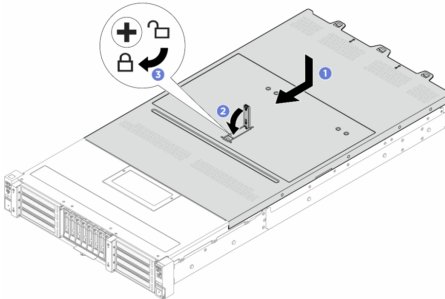
Figura 245. Instalando a tampa superior
