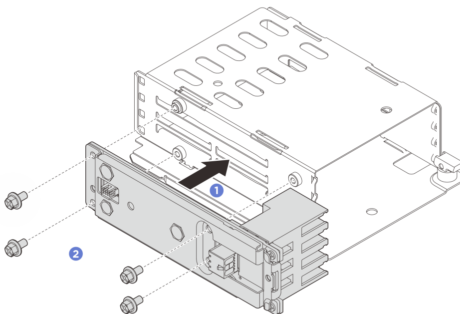
Figura 50. Instalação do conjunto de backplane
