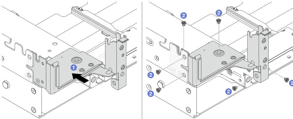
Figura 221. Instalação do suporte da parede traseira esquerda
