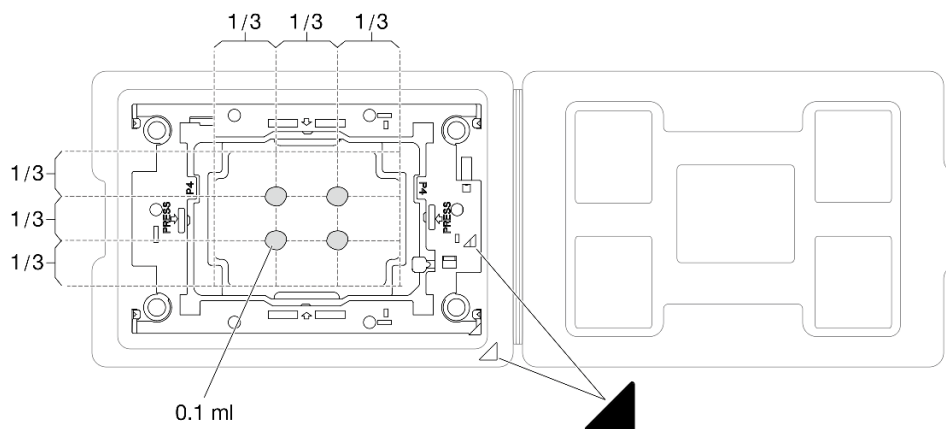
Figura 194. Aplicação de graxa térmica com processador na bandeja de remessa
