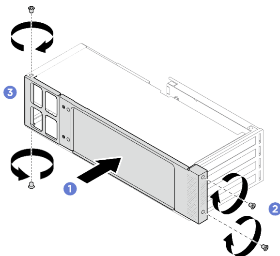
Figura 59. Instalação do suporte de apoio lateral
