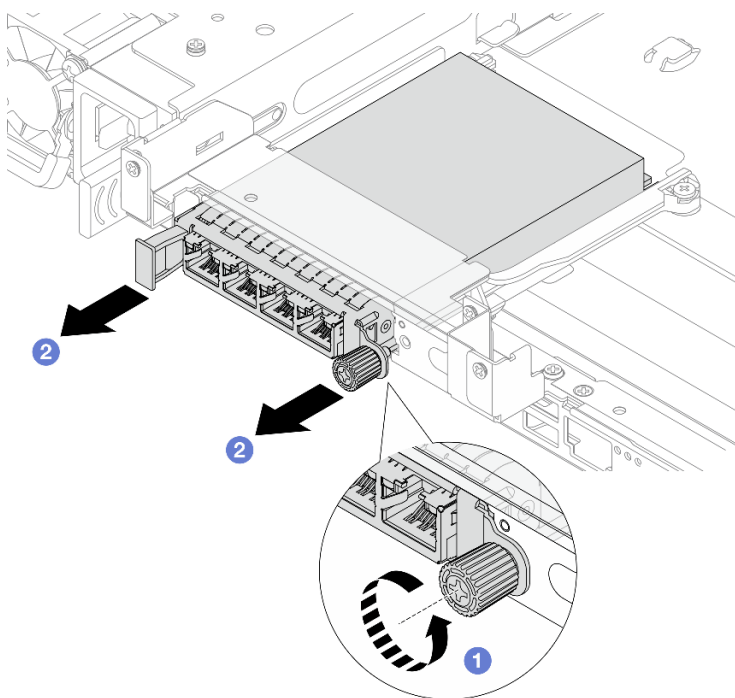
Figura 208. Removendo o módulo OCP traseiro
