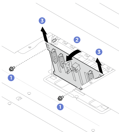
Figura 22. Removendo o backplane da unidade de 2,5 polegadas
