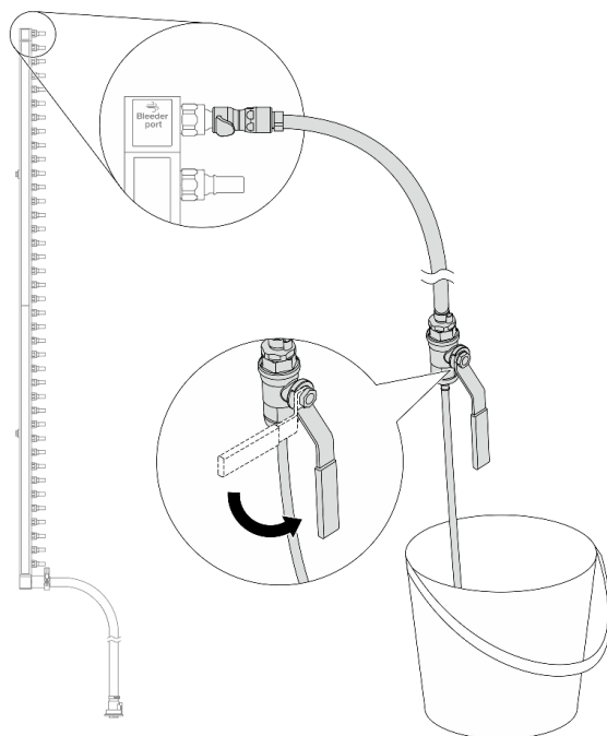
Figura 167. Abrindo a válvula de drenagem
