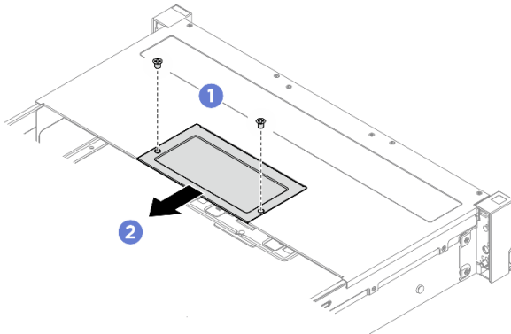
Figura 21. Removendo a placa da tampa
