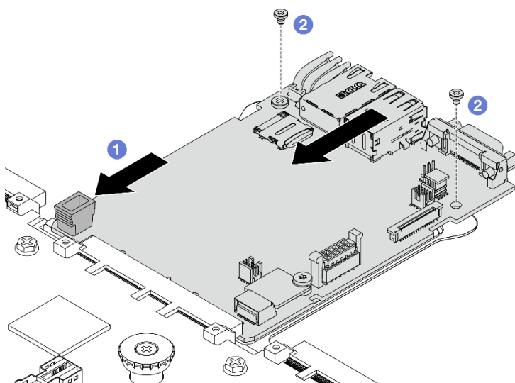
Figura 233. Instalando a placa de E/S do sistema na placa do processador
