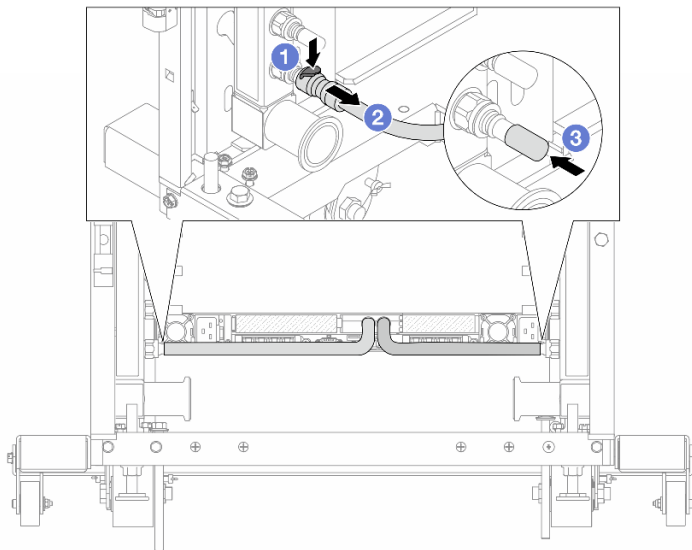
Figura 141. Remoção dos plugues de conexão rápida
