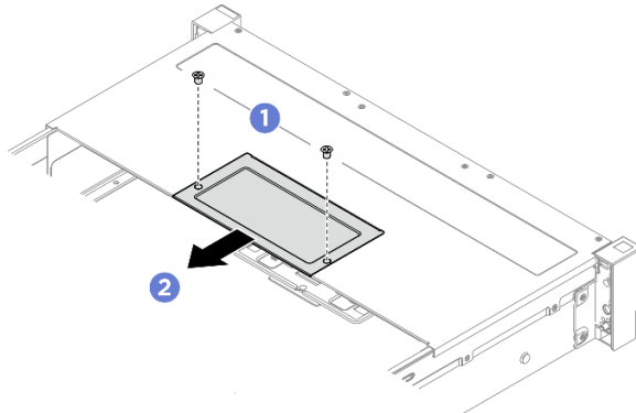
Figura 75. Removendo a placa da tampa
