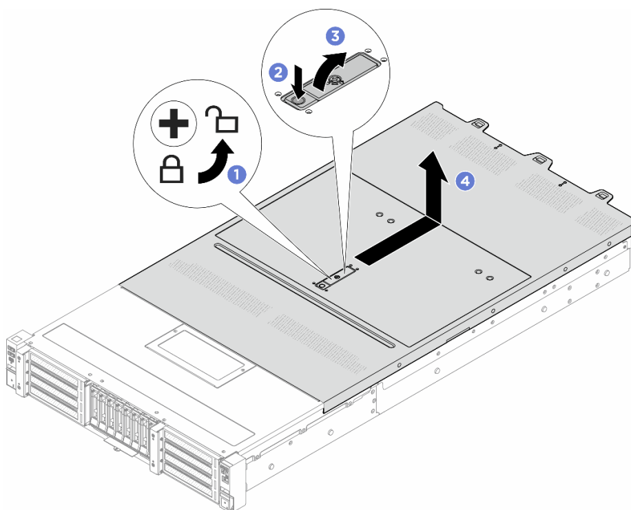
Figura 243. Removendo a tampa superior
