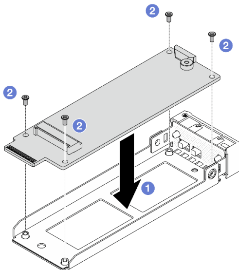
Figura 115. Instalando a placa de interposição M.2
