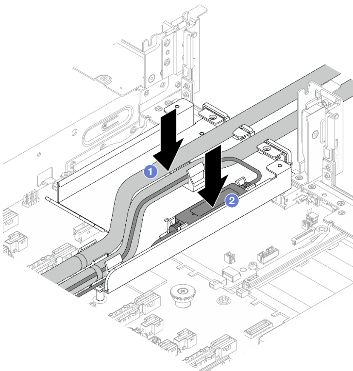
Figura 100. Colocação de mangueiras e módulo do sensor de detecção de líquidos
