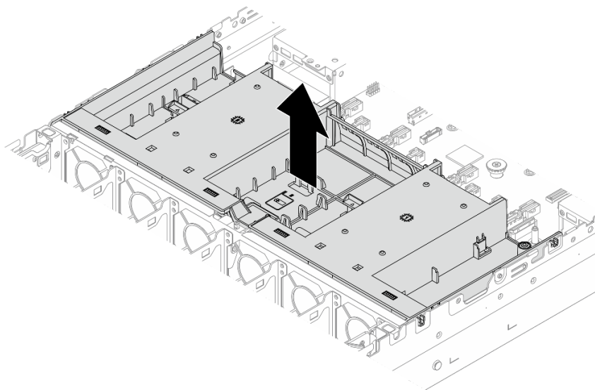
Figura 27. Removendo o defletor de ar
