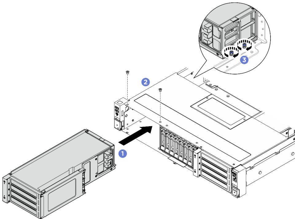
Figura 60. Instalação de conjunto de placa riser frontal
