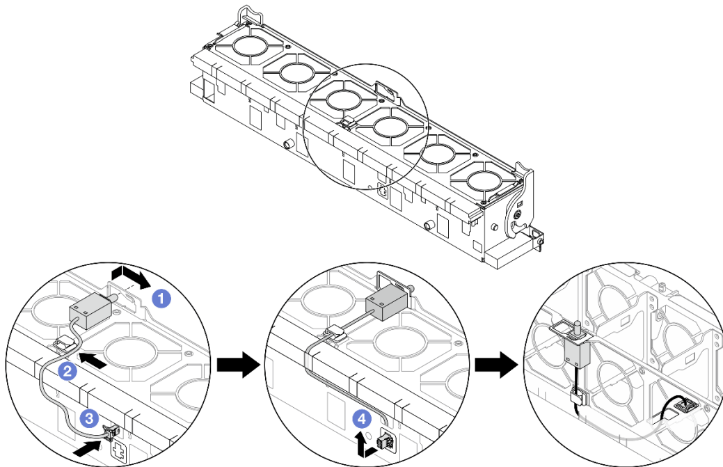
Figura 88. Instalando a chave de intrusão
