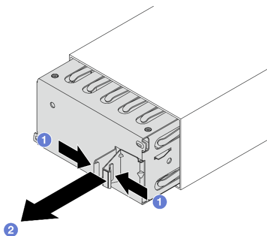
Figura 72. Remoção do preenchimento da unidade de fonte de alimentação
