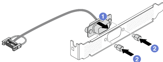
Figura 227. Montando o módulo de porta serial
