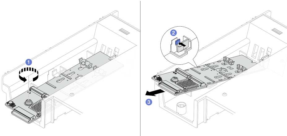
Figura 83. Removendo o backplane M.2 do defletor de ar
