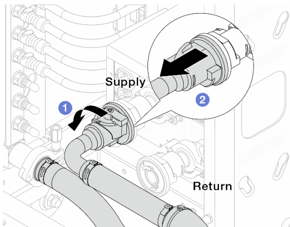
Figura 142. Removendo o conjunto de conexões
