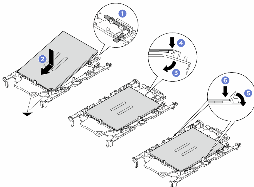
Figura 193. Instalando uma portadora de processador
