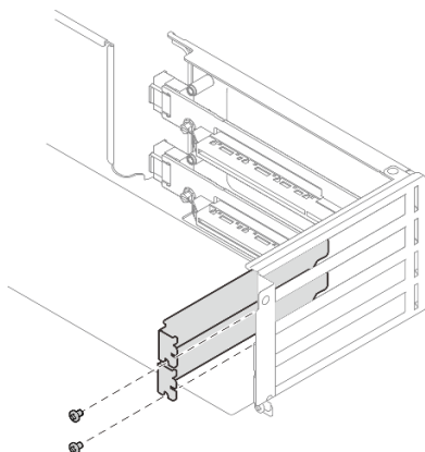
Figura 56. Preenchimento de slot PCIe
