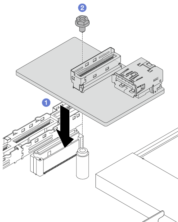
Figura 247. Instalando a placa de E/S USB
