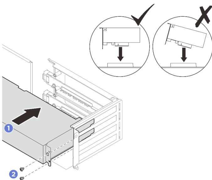
Figura 57. Instalação do adaptador PCIe
