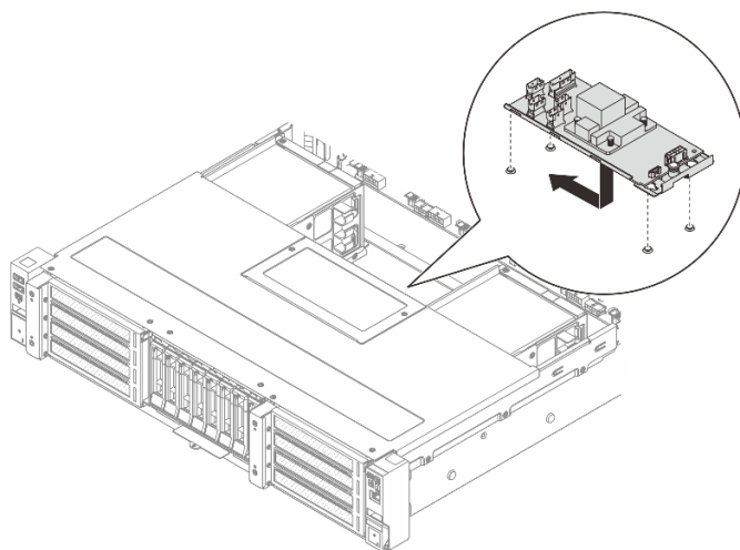
Figura 77. Instalação do adaptador CFF interno
