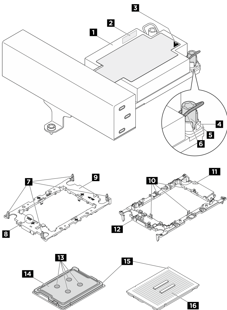
Figura 186. Componentes do PHM
