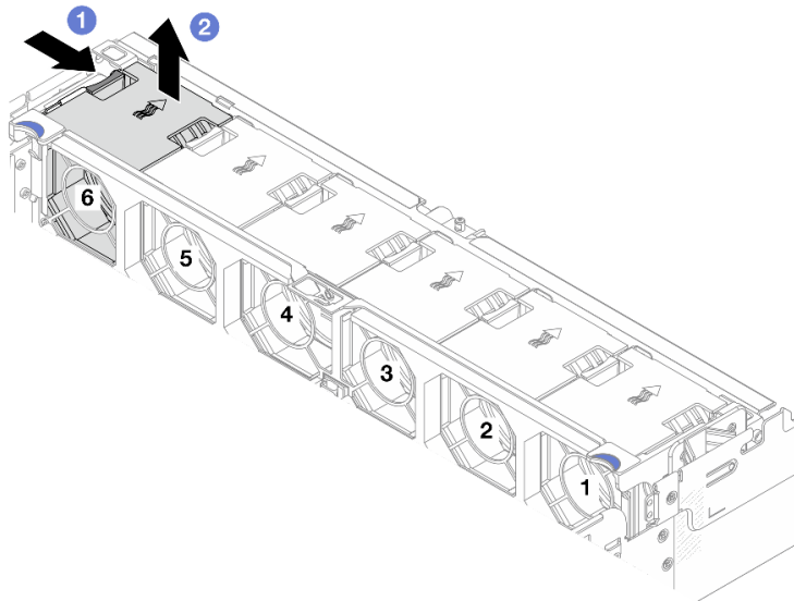
Figura 239. Removendo o ventilador do sistema
