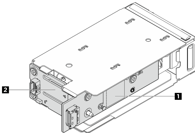
Figura 117. Backplanes da unidade M.2 frontal
