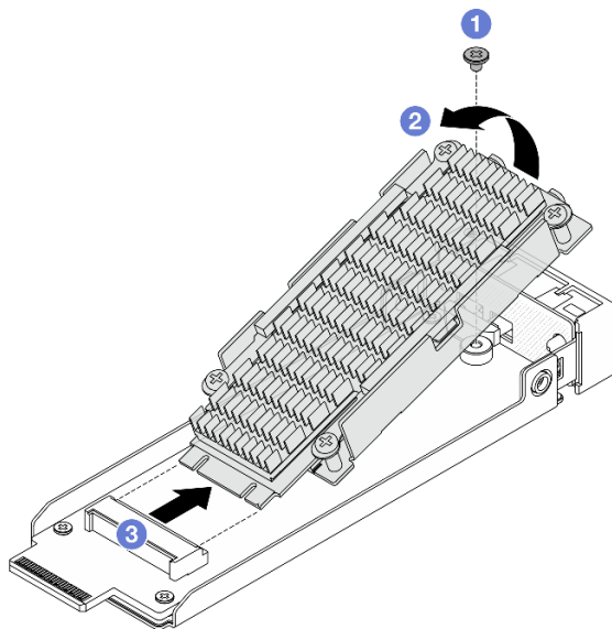
Figura 109. Remover a unidade M.2 com dissipador de calor
