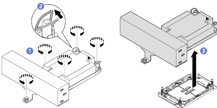
Figura 188. Remoção de um PHM de desempenho em forma de T de 1U
