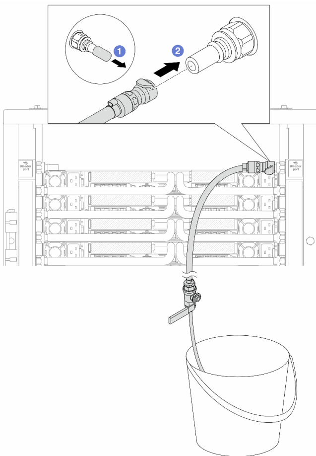
Figura 177. Instalando o kit de drenagem no lado de retorno
