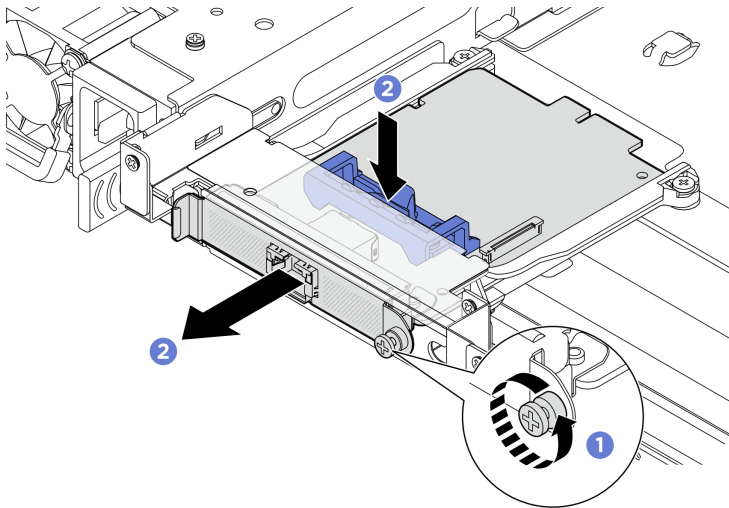
Figura 132. Removendo o adaptador NIC de gerenciamento
