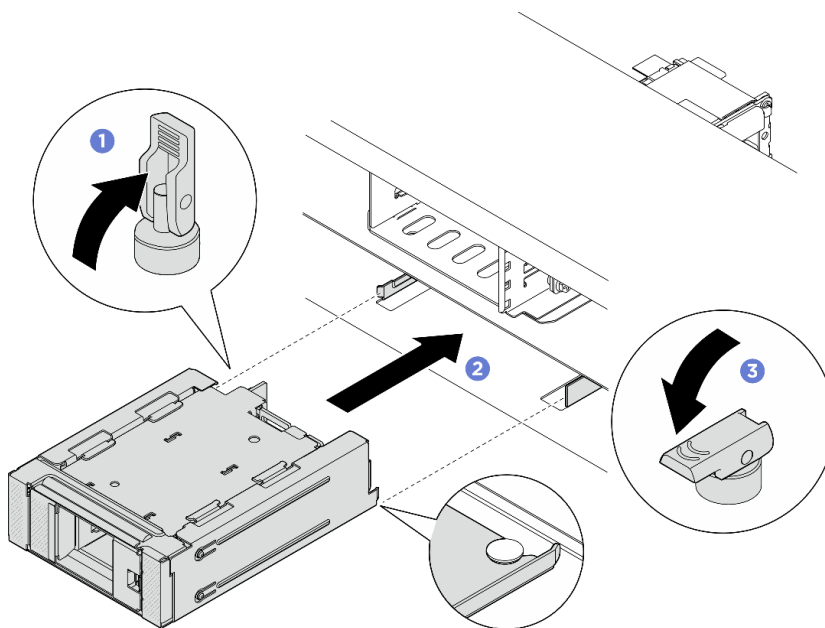
Figura 128. Instalação da gaiola de unidade M.2 frontal com quadro
