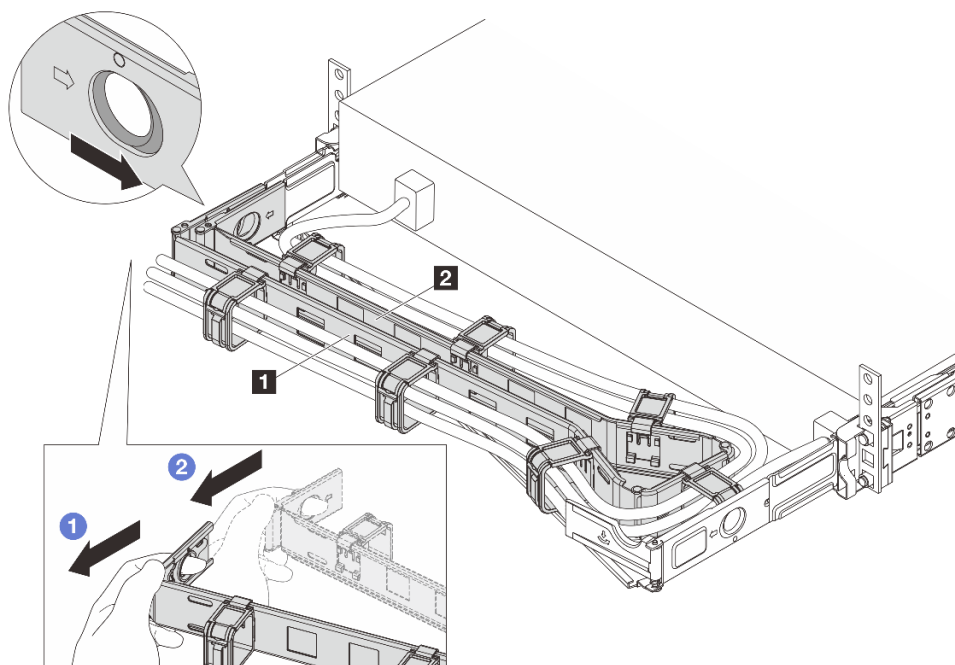
Figura 68. Removendo o lado esquerdo
