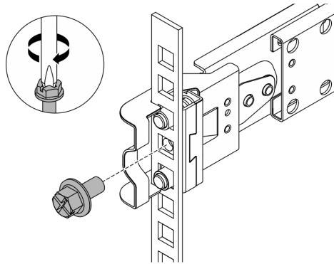
Figura 17. Fixando o servidor na parte traseira do rack
