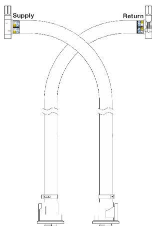
Figura 137. Kit de mangueira em linha 42U
