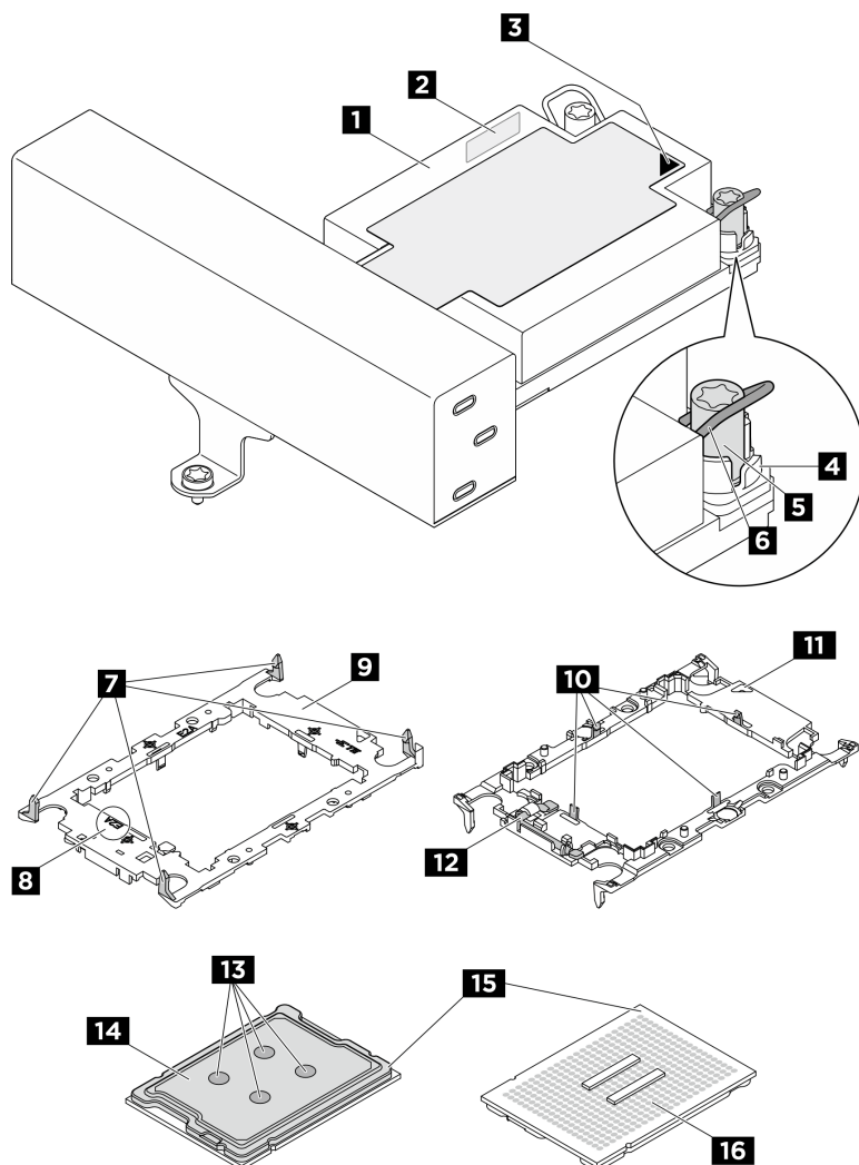
Figura 192. Componentes do PHM
