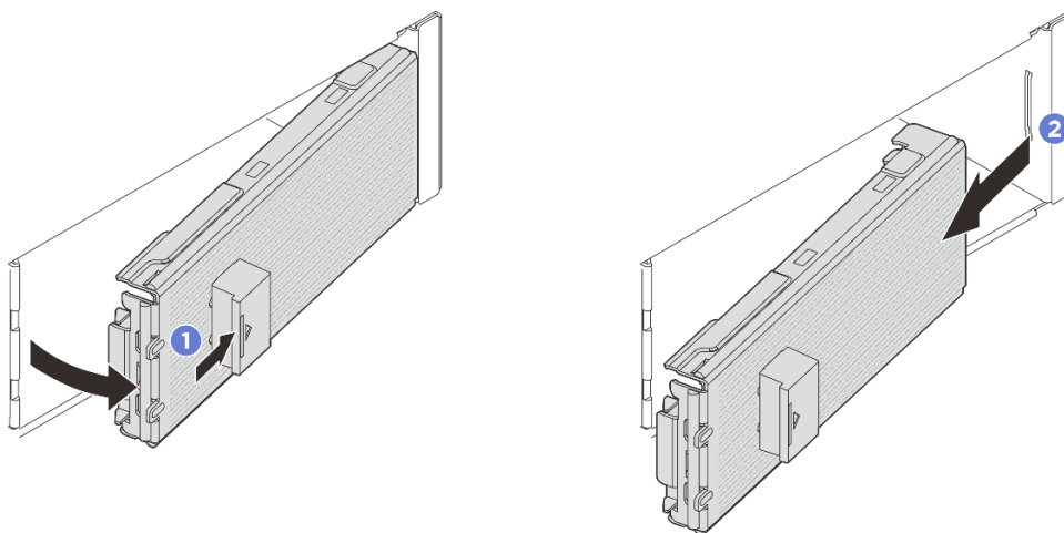
Figura 37. Remoção do painel E3.S
