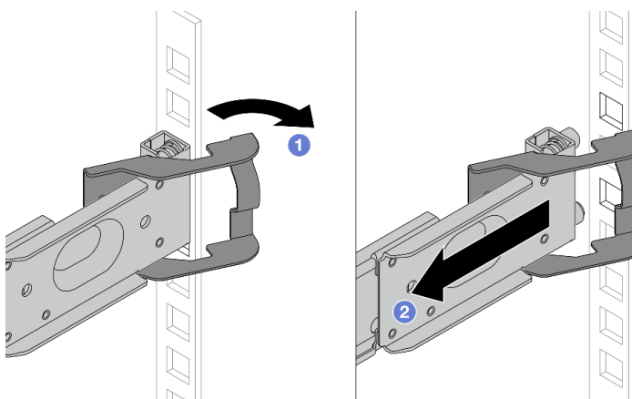
Figura 4. Removendo o trilho na parte traseira
