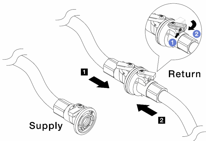
Figura 175. Abastecimento da instalação ao retorno do coletor
