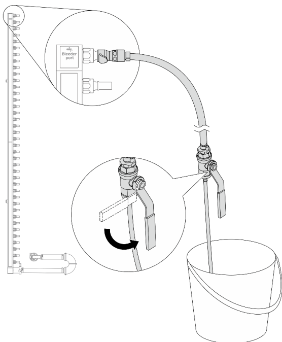
Figura 145. Abrindo a válvula de drenagem
