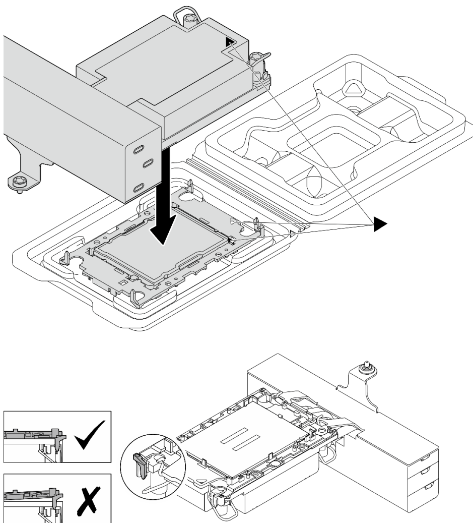
Figura 195. Montando o PHM com o processador na bandeja de remessa
