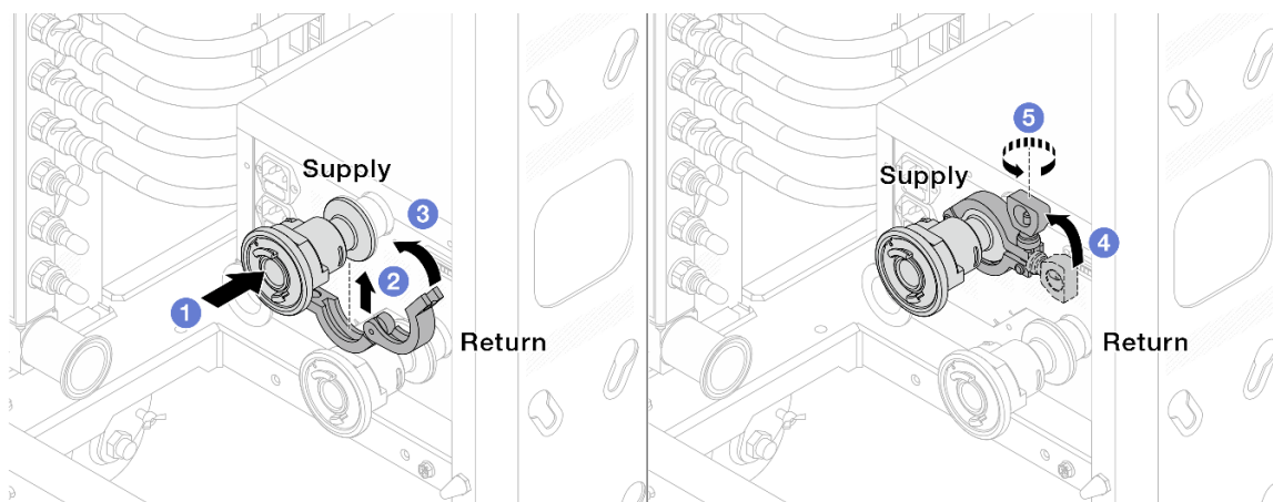
Figura 151. Instalando válvulas esféricas
