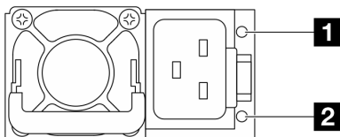
Figura 258. LEDs em uma unidade de fonte de alimentação CRPS Premium
