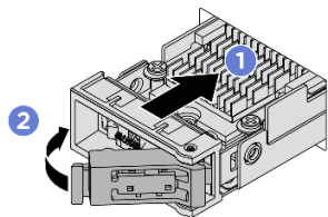
Figura 108. Instalação de um conjunto de unidade M.2
