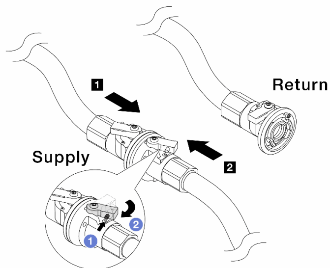
Figura 178. Abastecimento da instalação ao abastecimento do coletor
