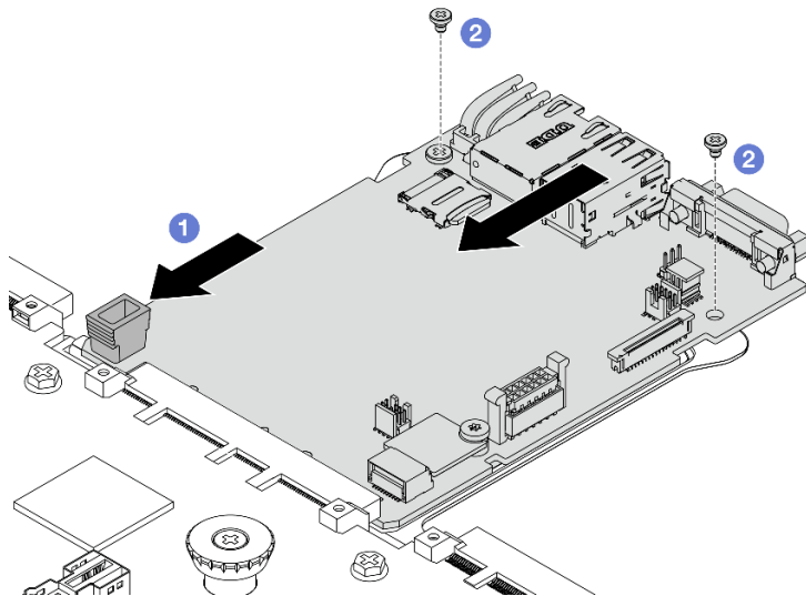
Figura 237. Instalando a placa de E/S do sistema na placa do processador
