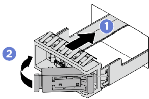
Figura 106. Instalação de uma bandeja da unidade M.2
