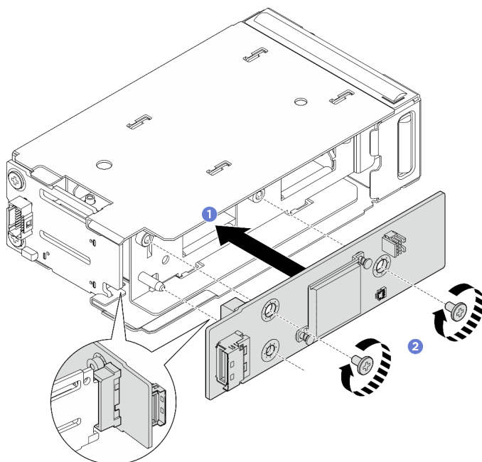
Figura 126. Instalação da placa do controlador M.2 frontal
