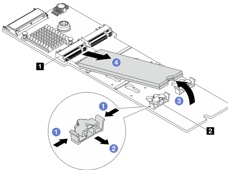
Figura 78. Removendo a unidade M.2
