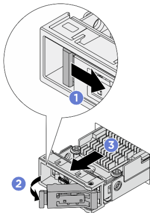
Figura 105. Remoção de um conjunto de unidade hot-swap M.2
