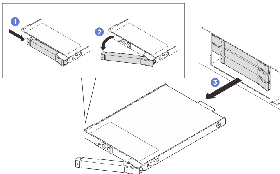
Figura 38. Remoção de uma unidade hot-swap E3.S
