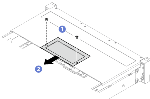
Figura 45. Remoção da placa de cobertura
