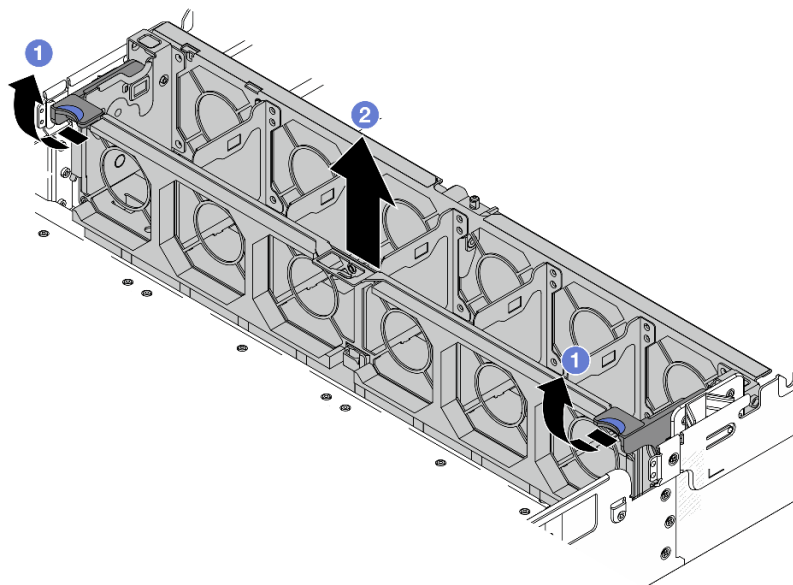
Figura 241. Removendo a gaiola do ventilador do sistema
