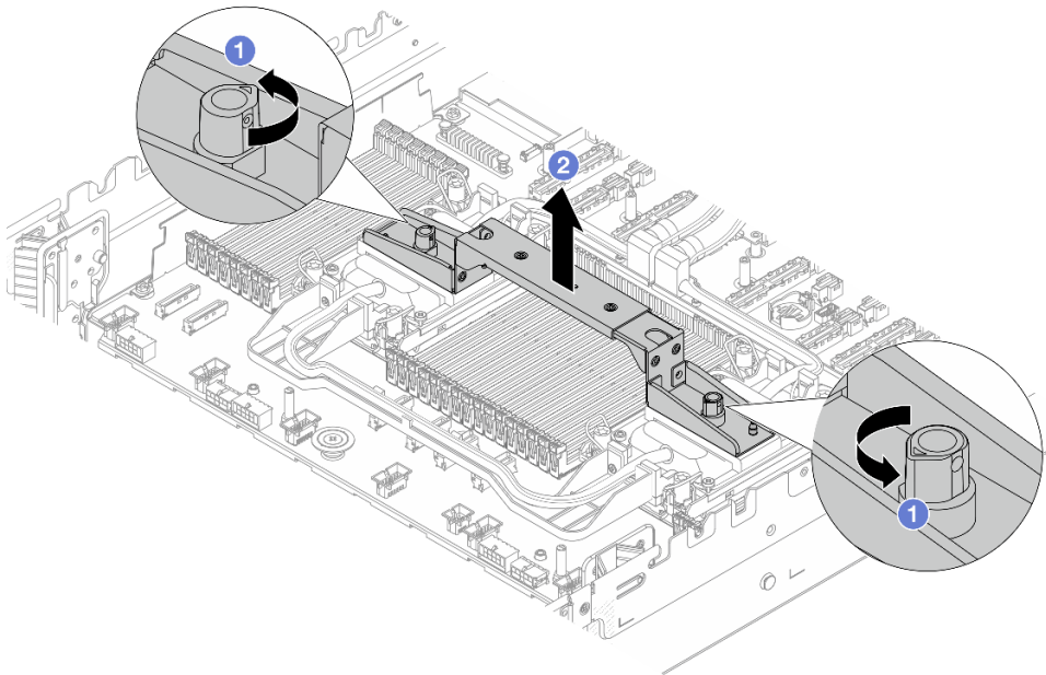
Figura 98. Removendo a alça do módulo
