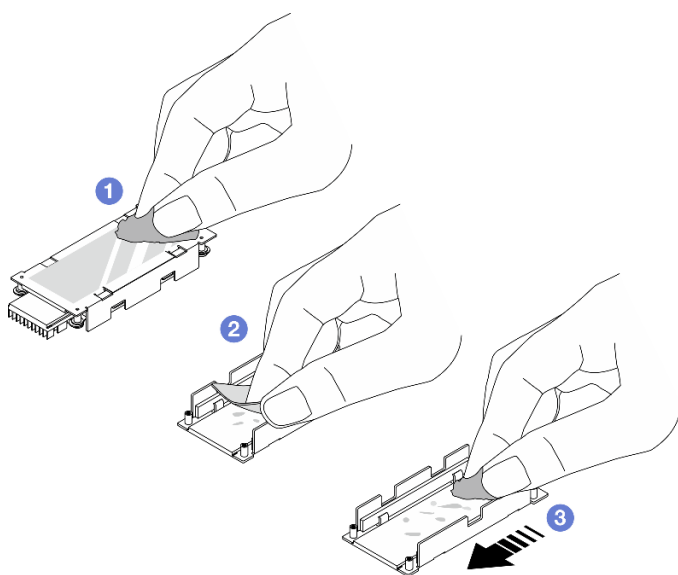
Figura 112. Limpeza do dissipador de calor e da placa inferior
