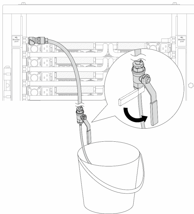
Figura 176. Abrindo a válvula de drenagem no lado de abastecimento
