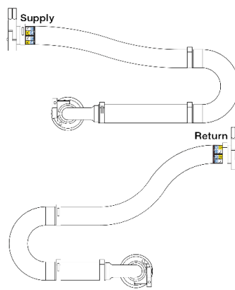
Figura 139. Conjunto de conexões em rack 48U
