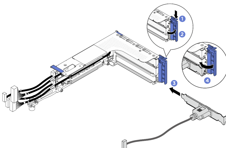
Figura 228. Instalando o módulo de porta serial
