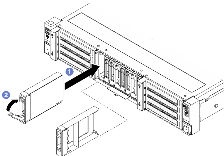
Figura 20. Instalando uma unidade hot-swap de 2,5"
