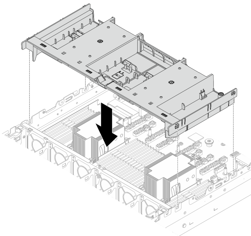
Figura 31. Instalando a placa defletora de ar
