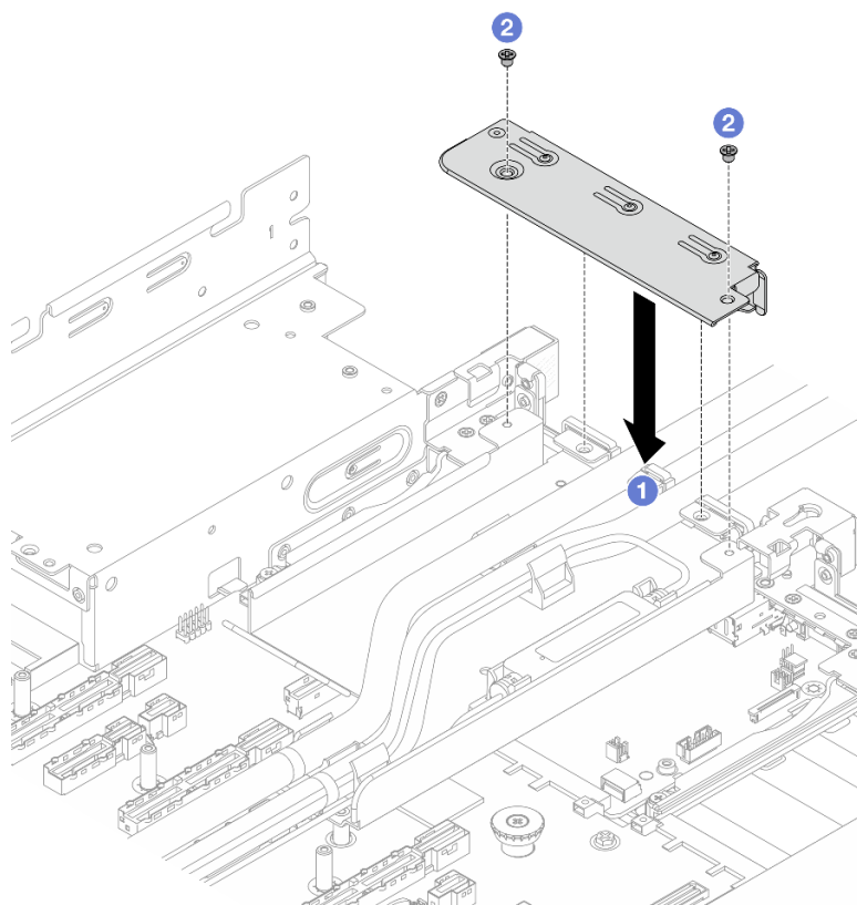
Figura 102. Instalação do suporte 1FH
