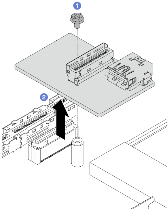
Figura 246. Removendo a placa de E/S USB
