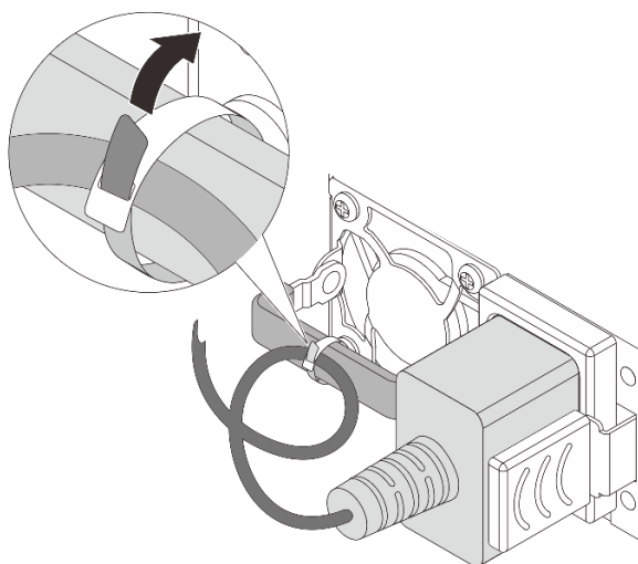
Figura 74. Roteamento e amarração do cabo de alimentação
