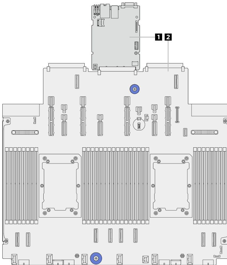
Figura 230. Layout do conjunto de placa-mãe
