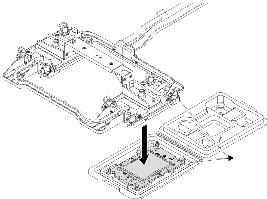
Figura 95. Instalando o processador
