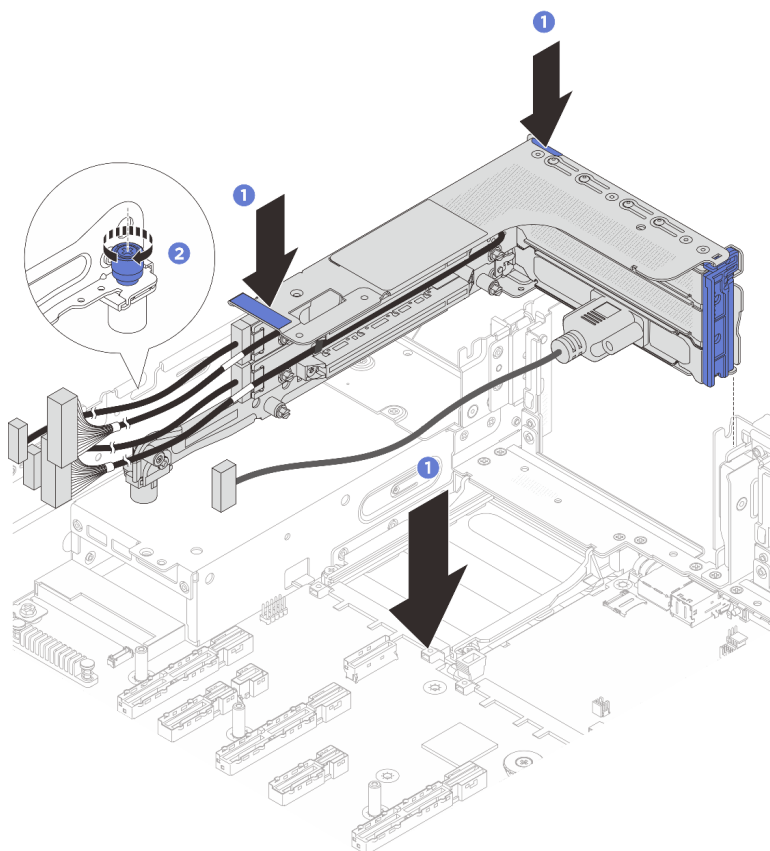
Figura 229. Instalando o conjunto de placa riser
