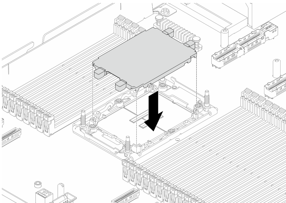
Figura 96. Instalação da tampa do soquete do processador
