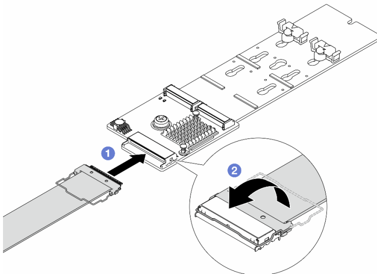
Figura 85. Conectando o cabo M.2
