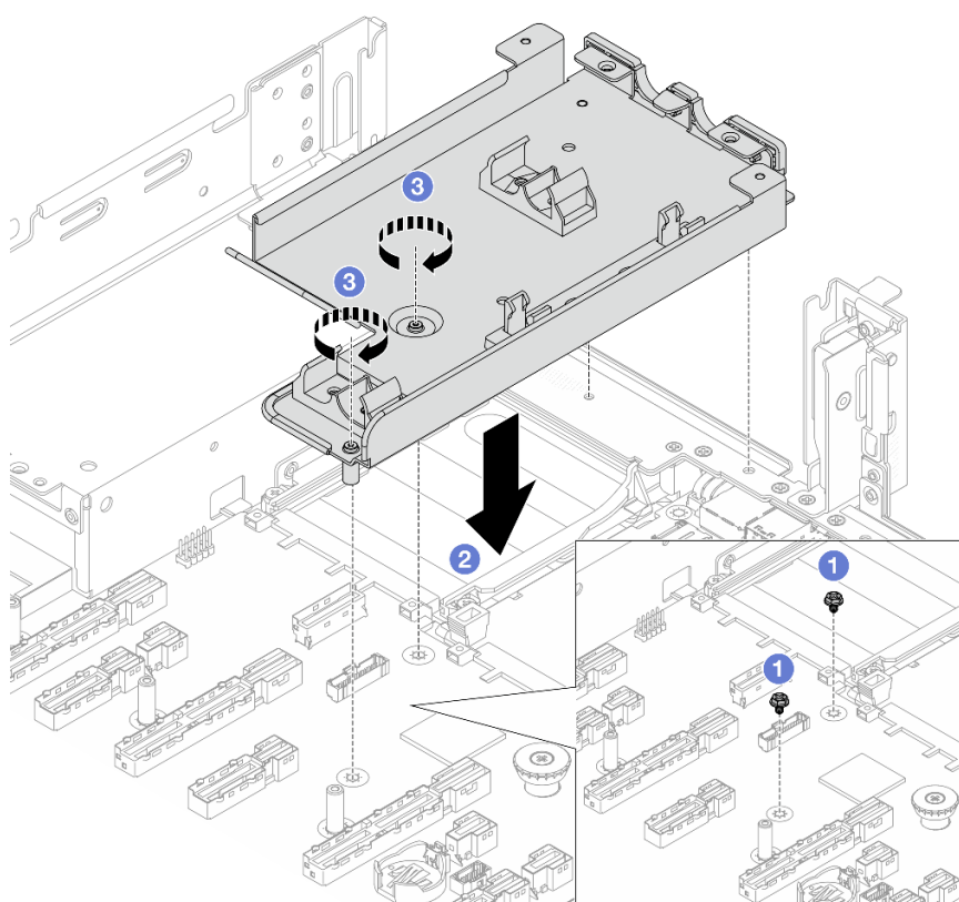
Figura 94. Instalando o suporte da mangueira
