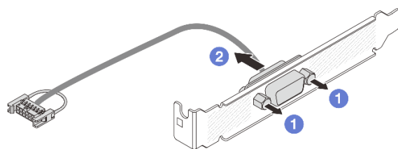
Figura 226. Desmontando o módulo de porta serial
