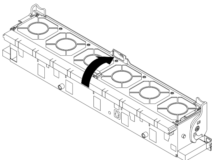
Figura 86. Girando o compartimento do ventilador
