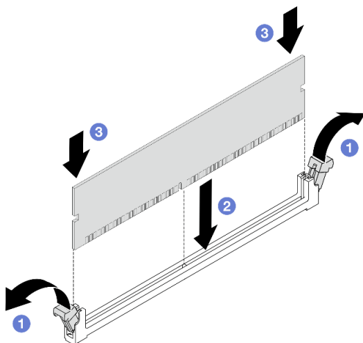
Figura 183. Instalando o módulo de memória
