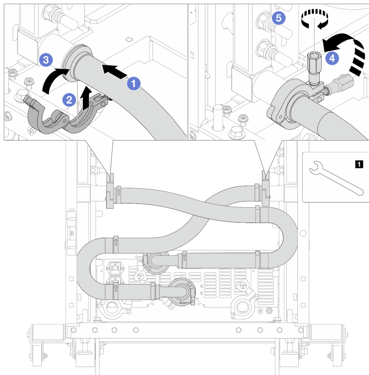
Figura 152. Instalando o conjunto de conexões
