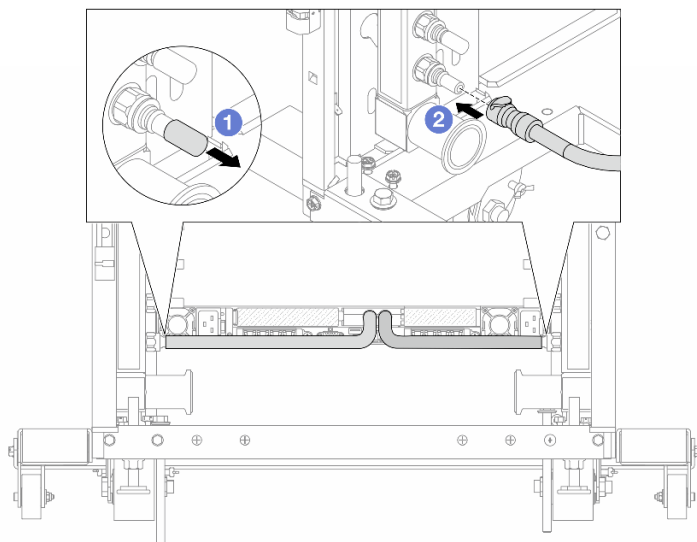
Figura 156. Instalando o plug de conexão rápida
