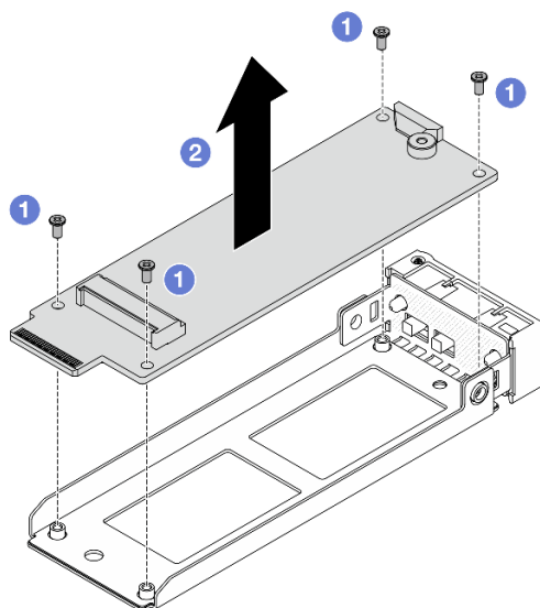
Figura 110. Removendo a placa de interposição M.2
