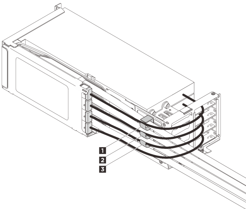
Figura 58. Clipes de cabos do conjunto de placa riser frontal
