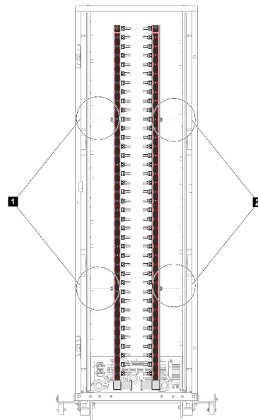
Figura 135. Coletores em um sistema em rack 42U
