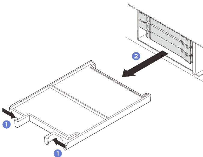
Figura 40. Remoção de um preenchimento de compartimentos
