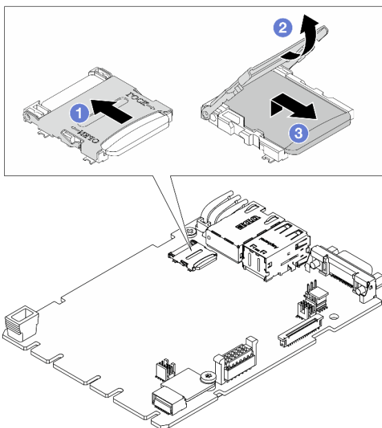
Figura 184. Removendo o cartão MicroSD
