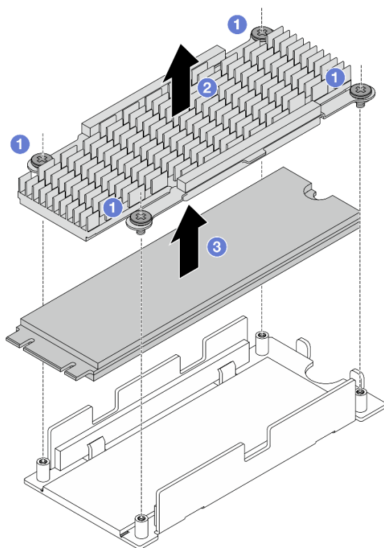
Figura 111. Removendo a unidade M.2
