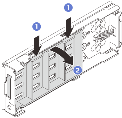
Figura 43. Remoção da placa interna
