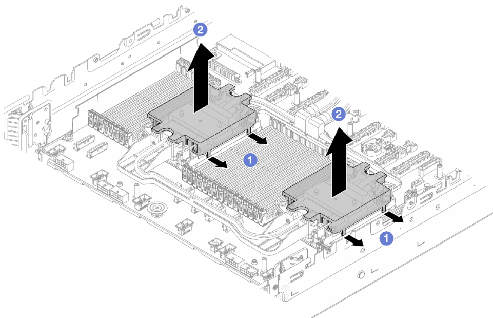
Figura 264. Removendo a tampa da placa fria
