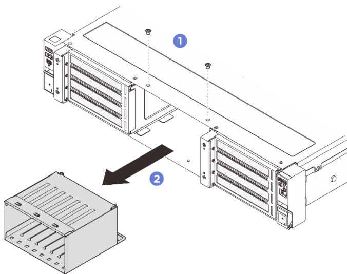
Figura 23. Remoção da gaiola da unidade de 2,5 polegadas
