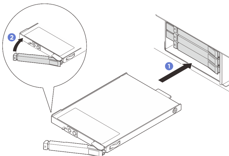
Figura 41. Instalação de uma unidade hot-swap E3.S
