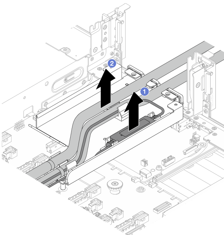
Figura 91. Desencaixe das mangueiras e módulo do sensor de detecção de líquidos
