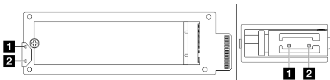
Figura 256. LEDs da placa de interposição M.2
