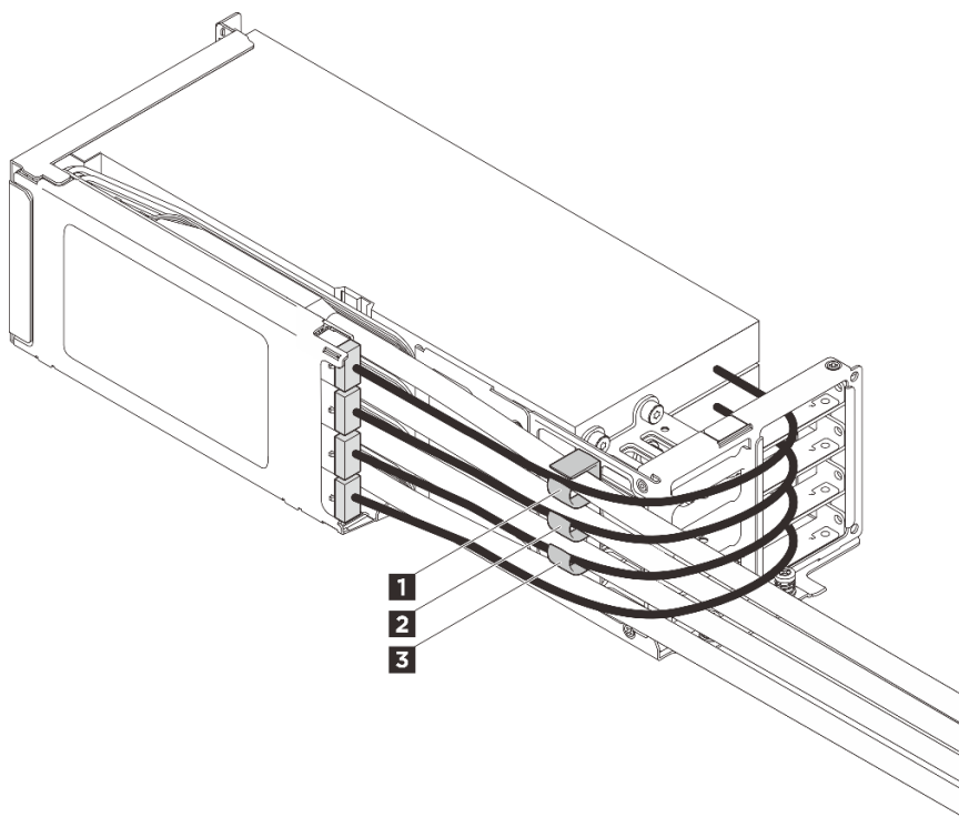
Figura 64. Cliques de cabos do conjunto de placa riser frontal
