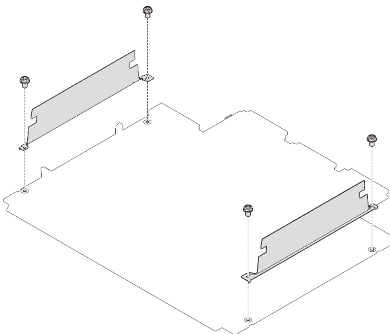
Figura 34. Instalação das parede de cabos
