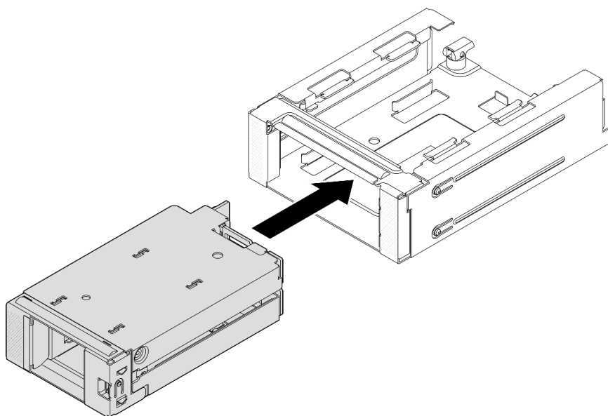
Figura 127. Instalação da gaiola de unidade M.2 frontal na estrutura da gaiola
