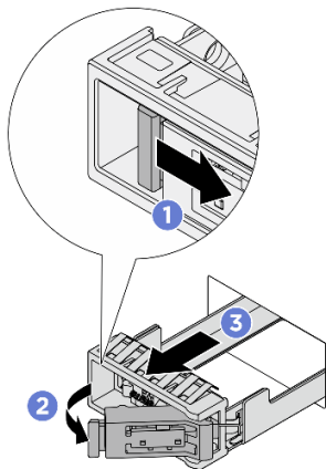
Figura 107. Remoção de uma bandeja da unidade M.2
