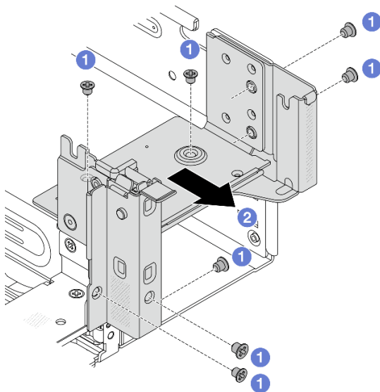
Figura 220. Remoção do suporte da parede traseira direita
