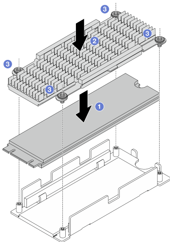
Figura 114. Instalando a unidade M.2
