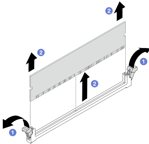
Figura 182. Removendo o módulo de memória
