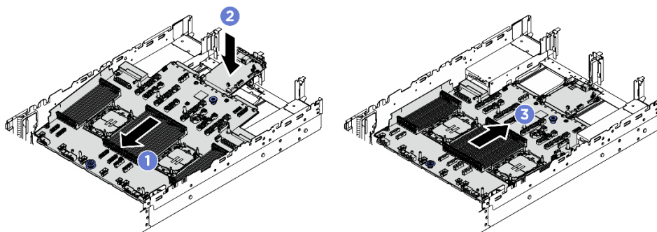
Figura 238. Instalando o conjunto de placa-mãe
