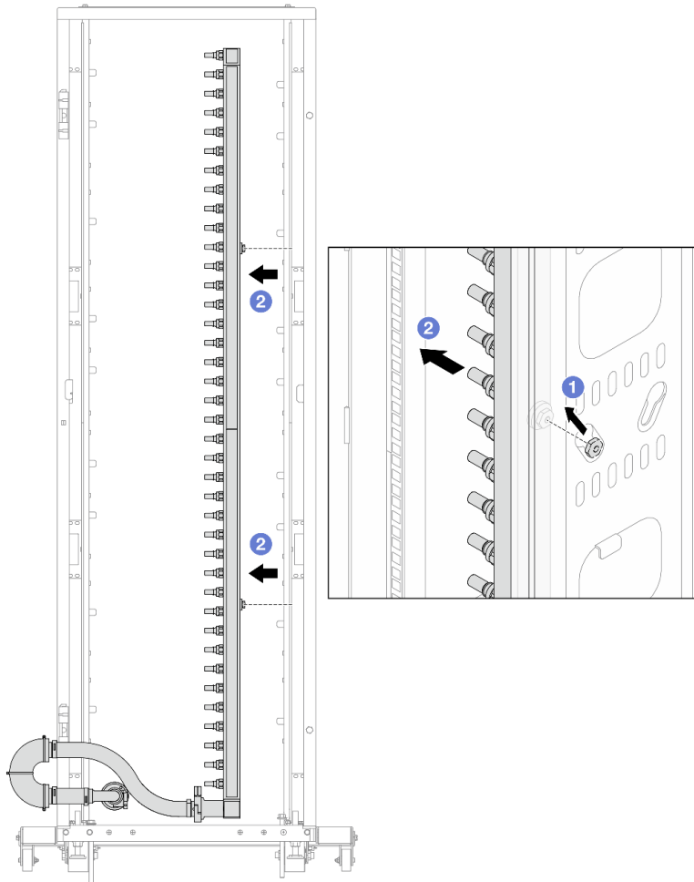
Figura 143. Removendo o coletor
