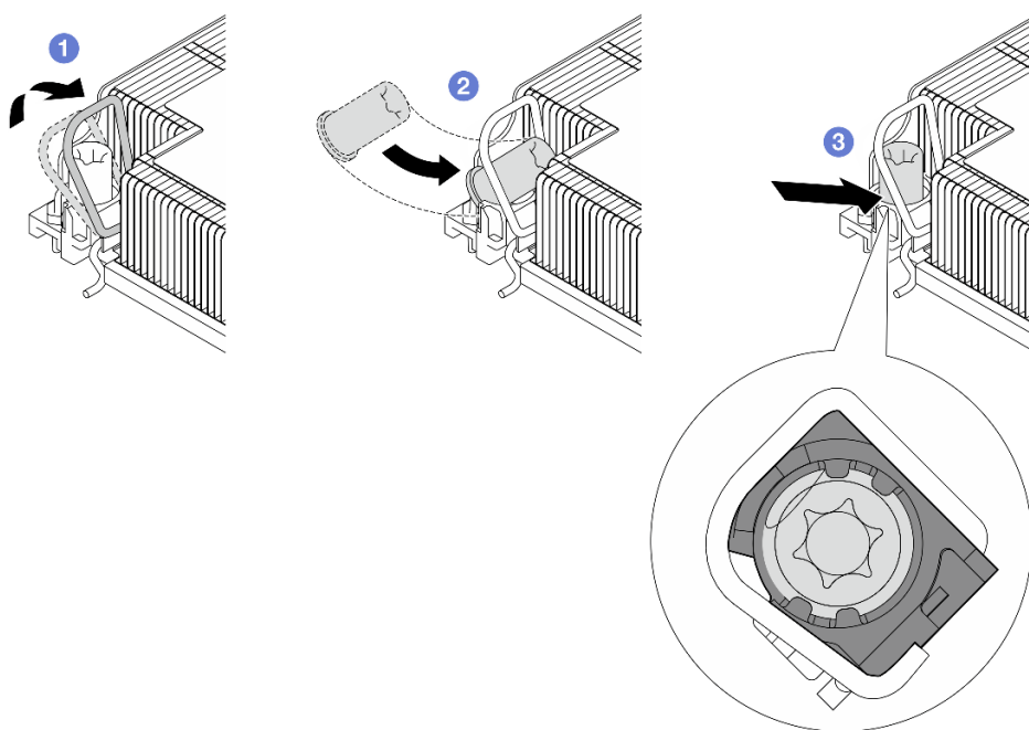
Figura 66. Instalando uma porca Torx T30 no dissipador de calor
