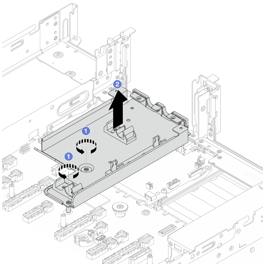
Figura 93. Removendo o suporte de mangueira
