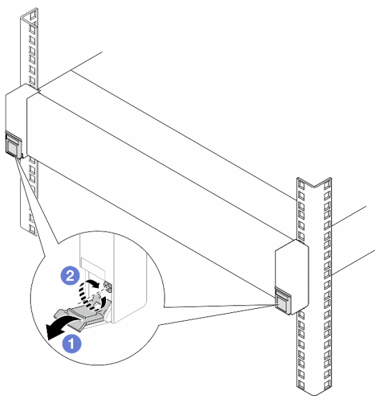
Figura 16. Fixando o servidor na parte frontal do rack
