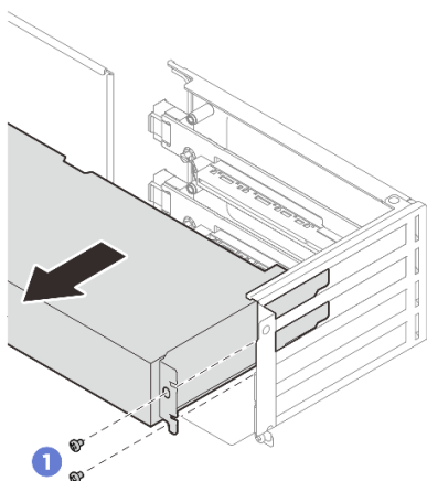
Figura 54. Remoção do adaptador PCIe
