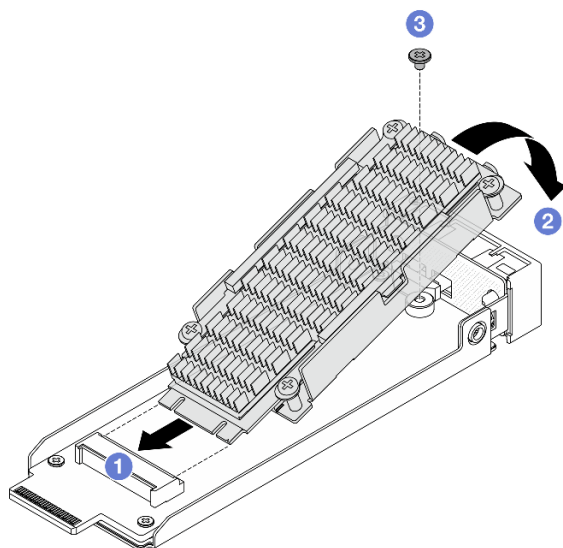
Figura 116. Instalação da unidade M.2 com dissipador de calor
