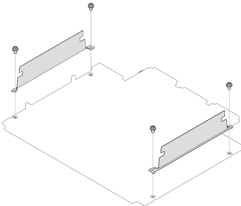
Figura 33. Remoção das paredes do cabo
