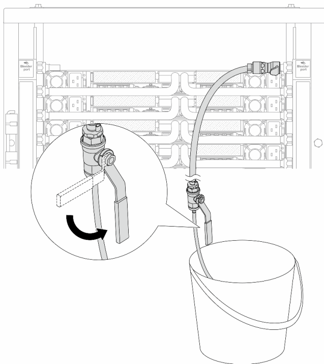
Figura 179. Abrindo a válvula de drenagem no lado de retorno
