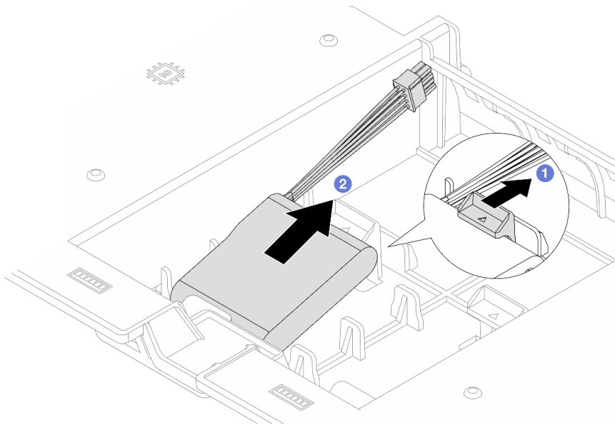
Figura 206. Removendo o módulo de energia flash RAID do defletor de ar
