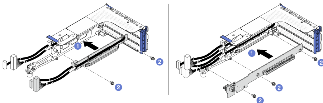
Figura 215. Instalação de placas riser na gaiola de placa riser 3FH
