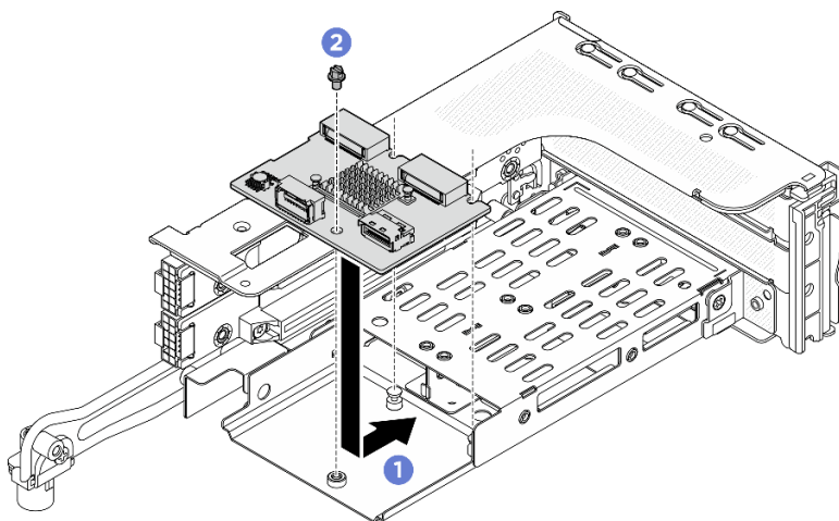
Figura 131. Instalação do backplane M.2 na gaiola da placa riser 3FH M.2
