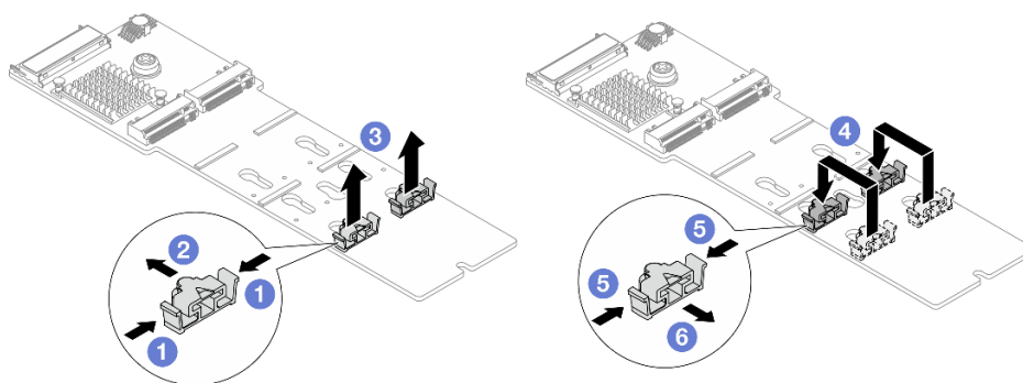
Figura 79. Ajustando o retentor M.2
