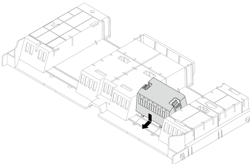
Figura 29. Instalando o preenchimento do defletor de ar
