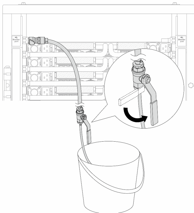
Figura 162. Abrindo a válvula de drenagem no lado de abastecimento
