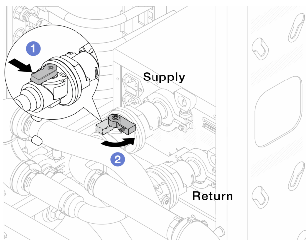
Figura 140. Fechando as válvulas esféricas
