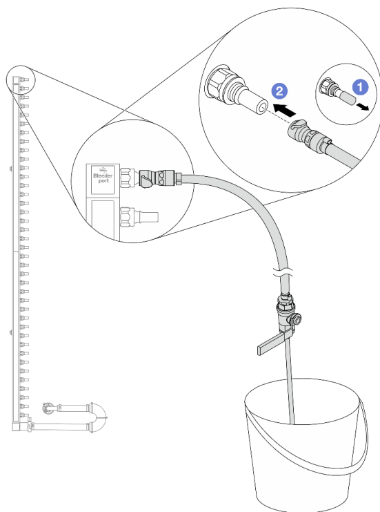
Figura 144. Instalando o kit de drenagem no lado de abastecimento
