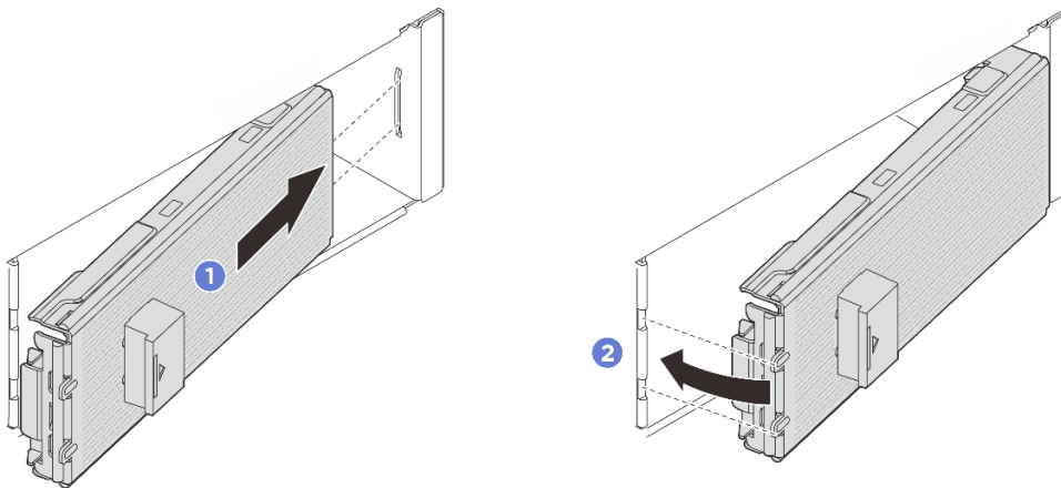
Figura 44. Instalação do painel E3.S
