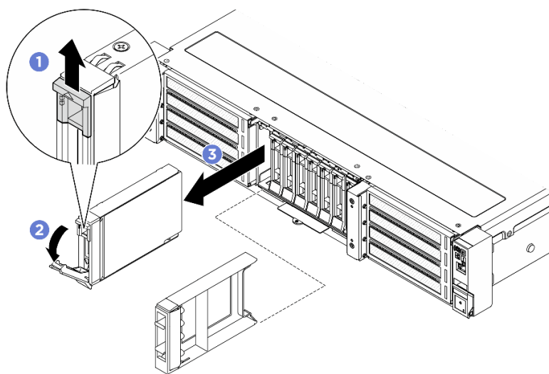
Figura 18. Removendo uma unidade hot-swap de 2,5 polegadas
