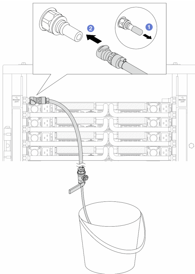
Figura 174. Instalando o kit de drenagem no lado de abastecimento
