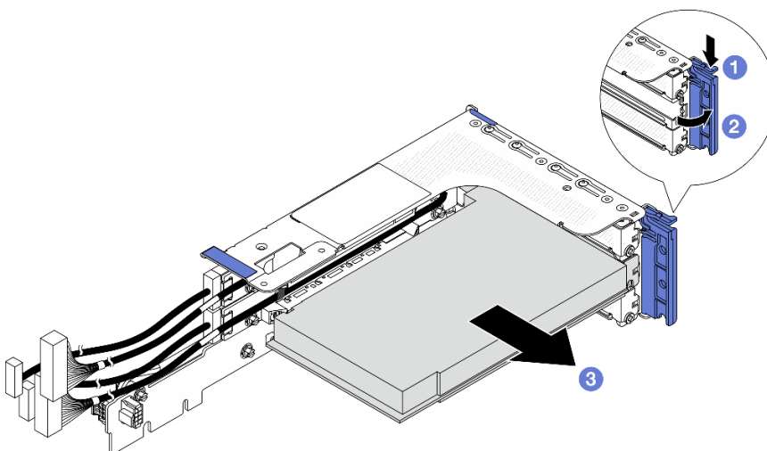
Figura 213. Remoção de um adaptador PCIe da gaiola da placa riser 3FH
