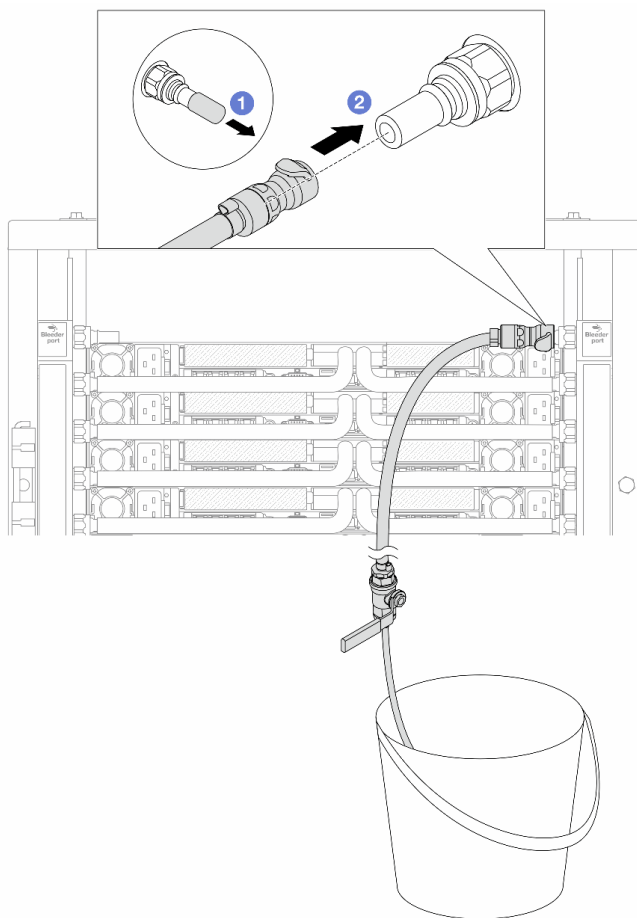
Figura 160. Instalando o kit de drenagem no lado de retorno
