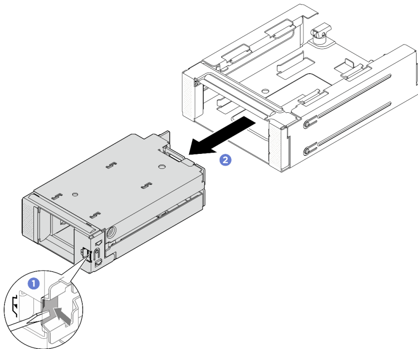
Figura 119. Remoção da gaiola de unidade M.2 frontal da estrutura
