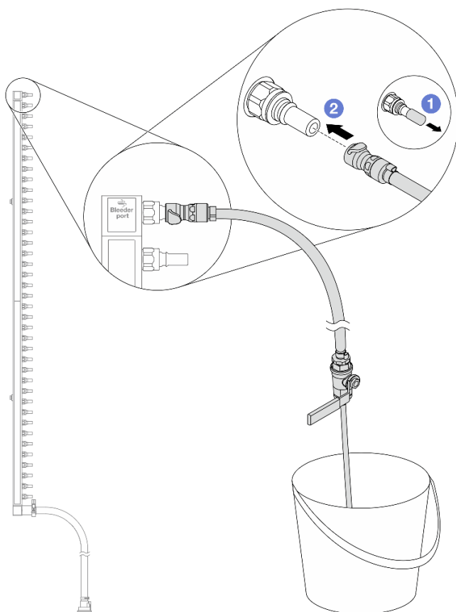
Figura 166. Instalando o kit de drenagem no lado de abastecimento
