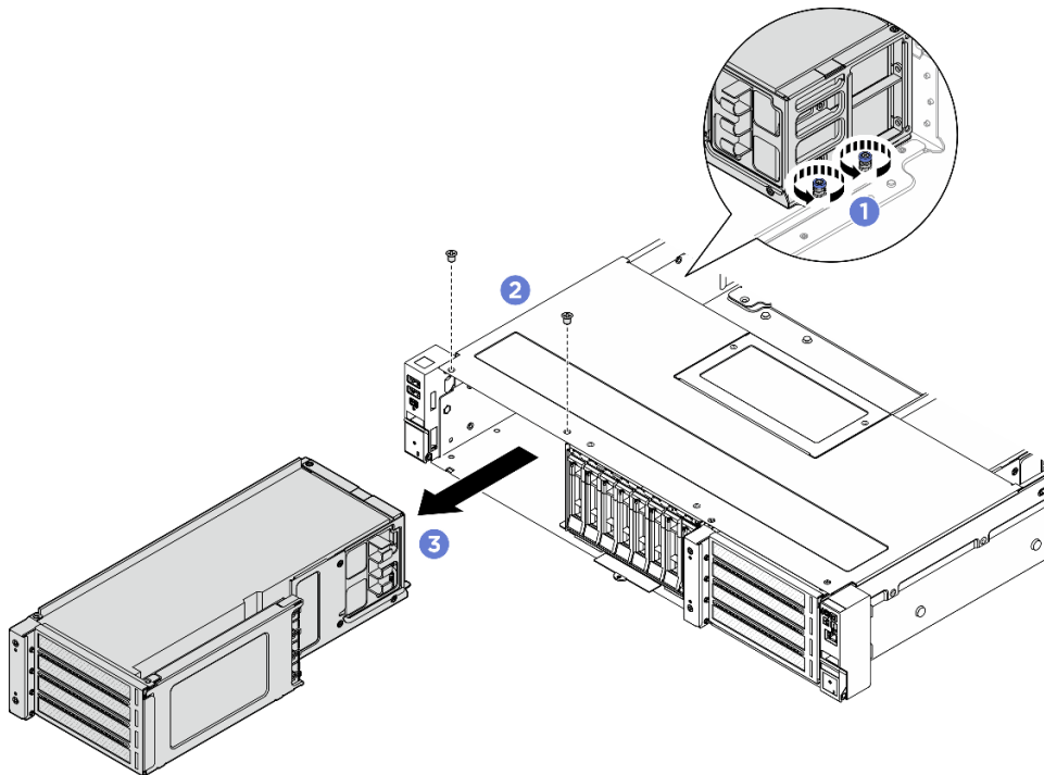
Figura 52. Remoção do conjunto de placa riser frontal
