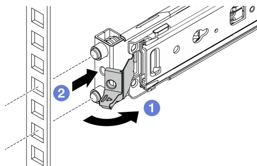
Figura 3. Removendo o trilho na parte frontal
