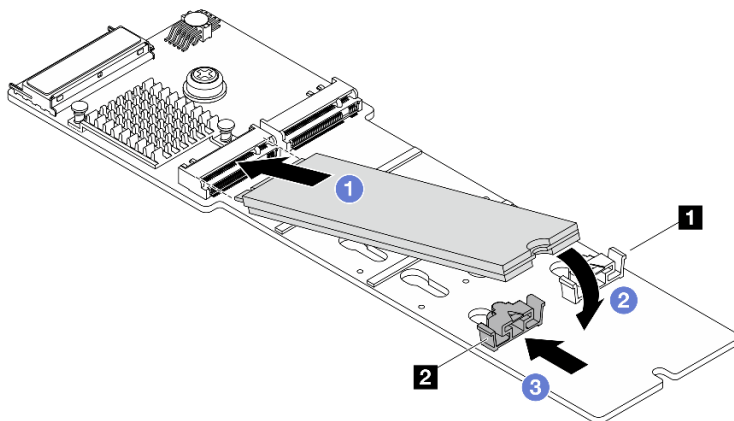
Figura 81. Instalando a unidade M.2
