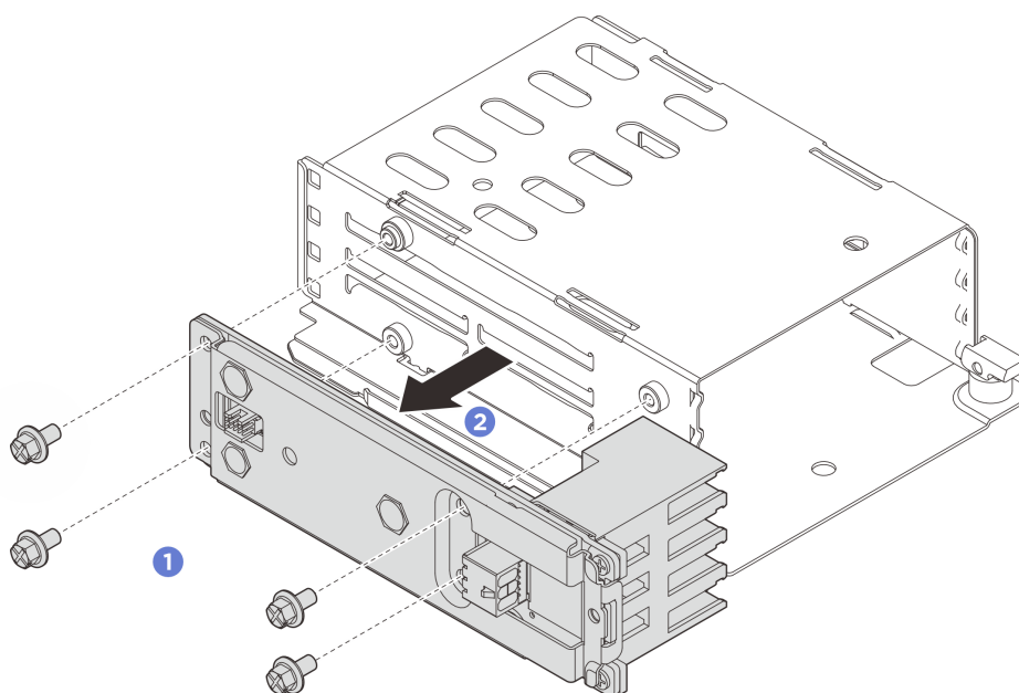
Figura 47. Remoção do conjunto de backplane
