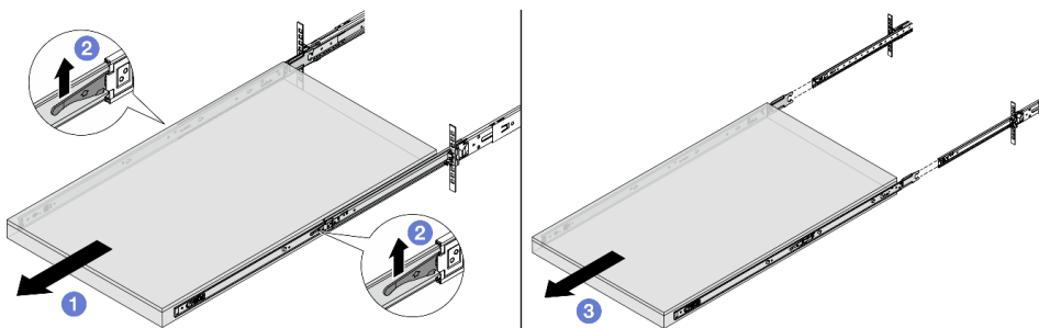
Figura 9. Puxando o servidor
