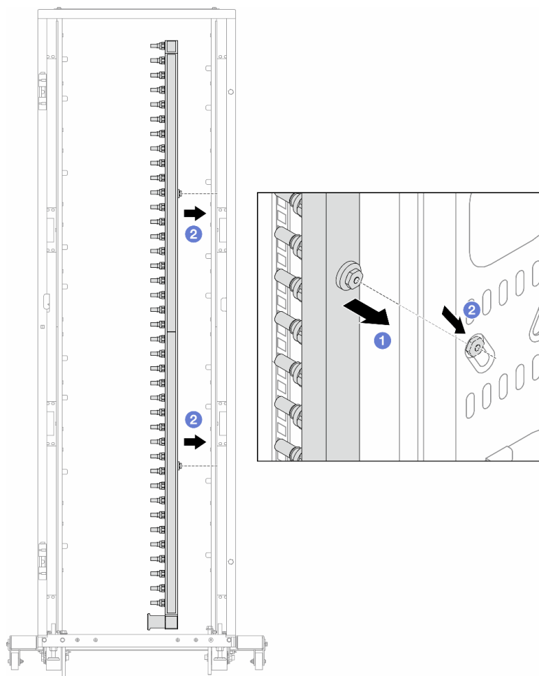
Figura 171. Instalando o coletor
