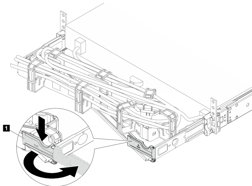
Figura 67. Ajustando o lado direito
