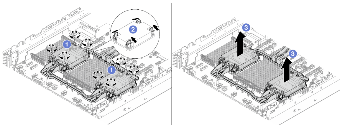
Figura 92. Removendo a Processor Neptune Core Module
