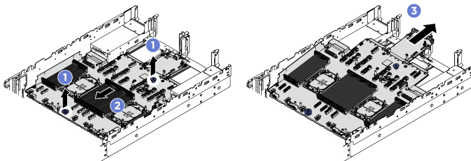
Figura 235. Removendo o conjunto de placa-mãe
