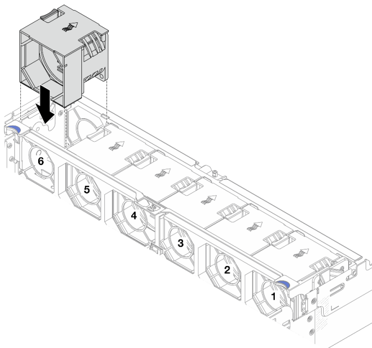
Figura 240. Instalando o ventilador do sistema
