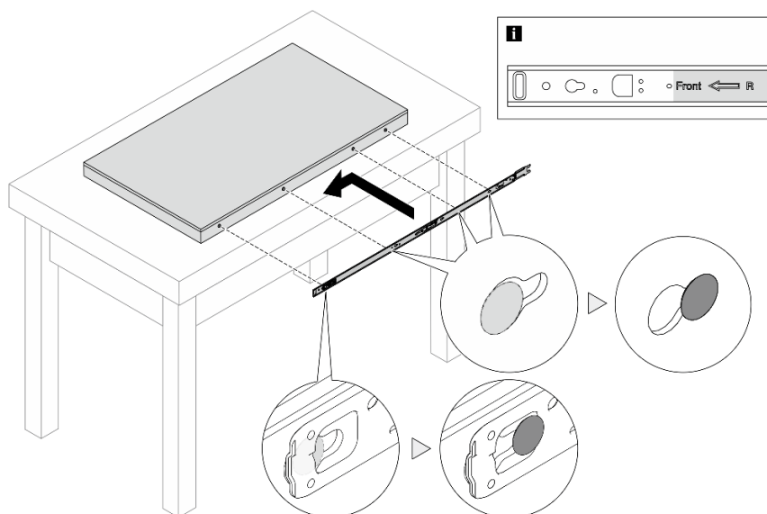
Figura 12. Instalando trilhos internos
