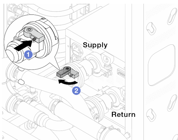
Figura 158. Abrindo as válvulas esféricas
