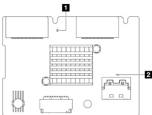
Figura 257. LEDs do backplane M.2 traseiro
