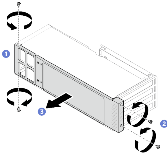
Figura 53. Remoção do suporte de apoio lateral
