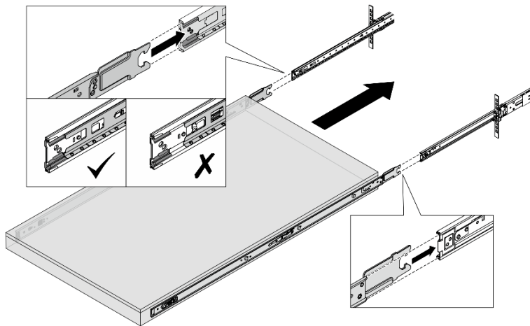
Figura 14. Trilhos de intertravamento
