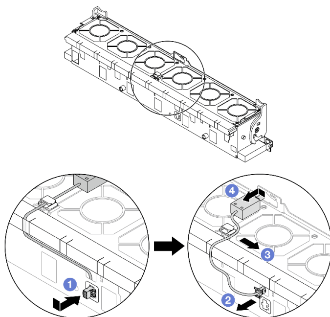
Figura 87. Removendo a chave de intrusão
