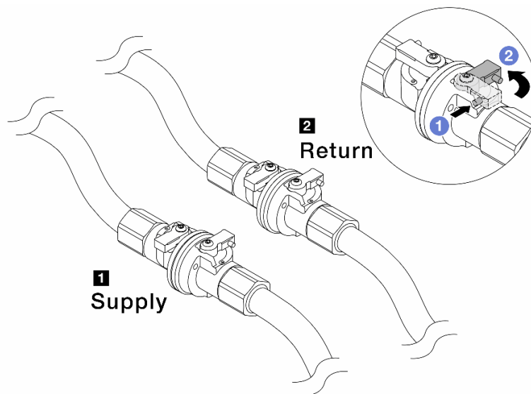
Figura 163. Fechando as válvulas esféricas
