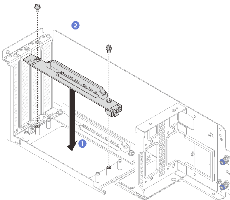
Figura 63. Instalação da placa riser
