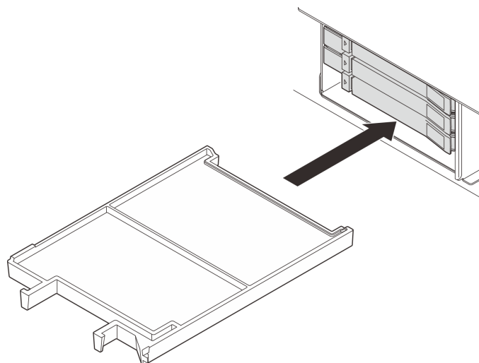
Figura 42. Instalação de um preenchimento de compartimentos
