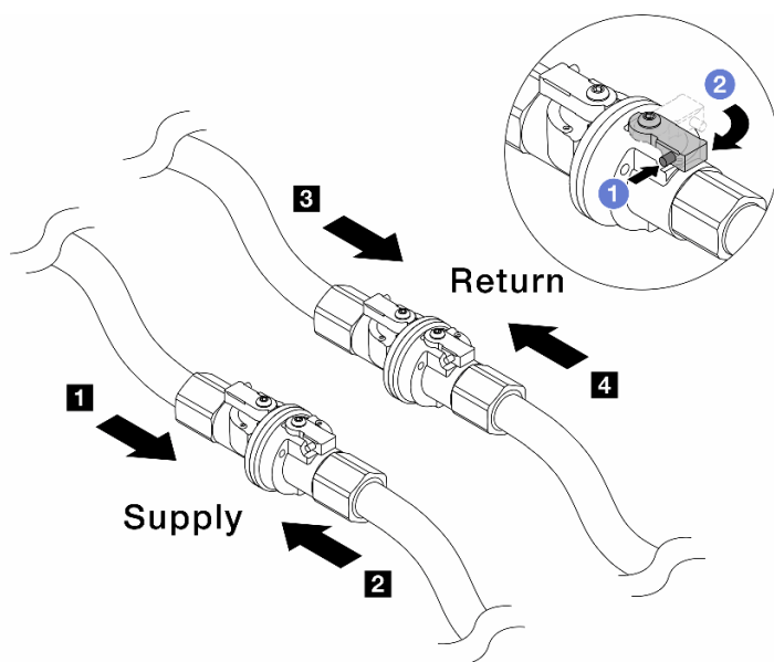
Figura 181. Abrindo as válvulas esféricas
