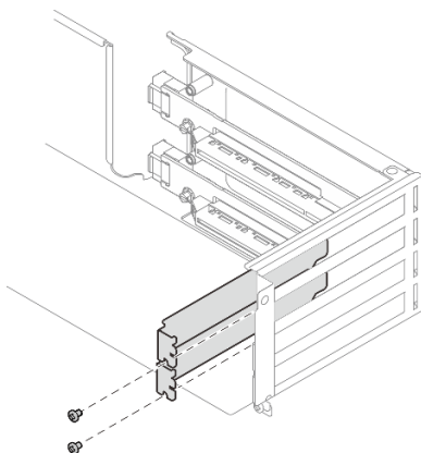
Figura 55. Preenchimento de slot PCIe
