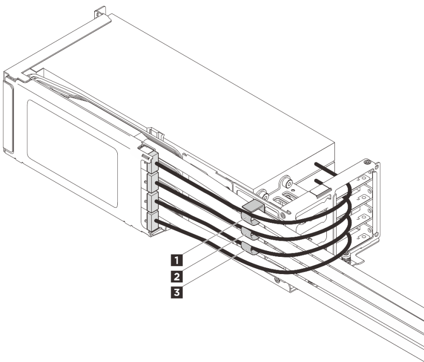
Figura 61. Clipes de cabos do conjunto de placa riser frontal
