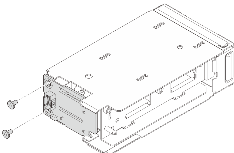
Figura 125. Instalação do backplane de inicialização M.2
