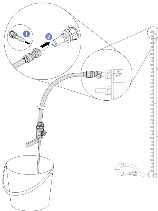
Figura 146. Instalando o kit de drenagem no lado de retorno
