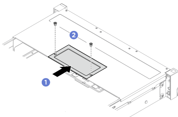
Figura 26. Instalação da placa de cobertura
