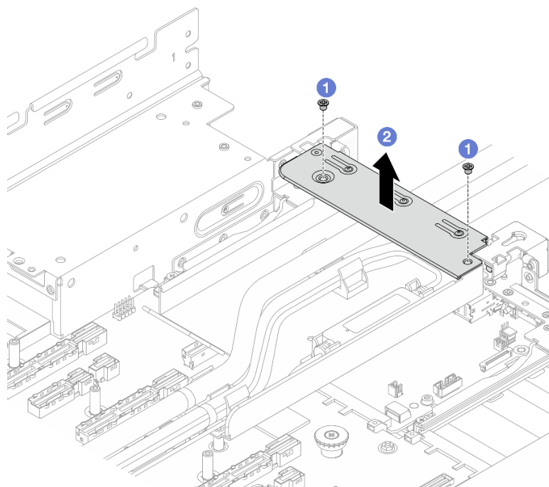
Figura 89. Remoção do suporte 1FH
