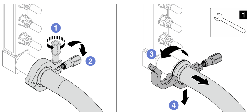
Figura 170. Separando o coletor do kit da mangueira
