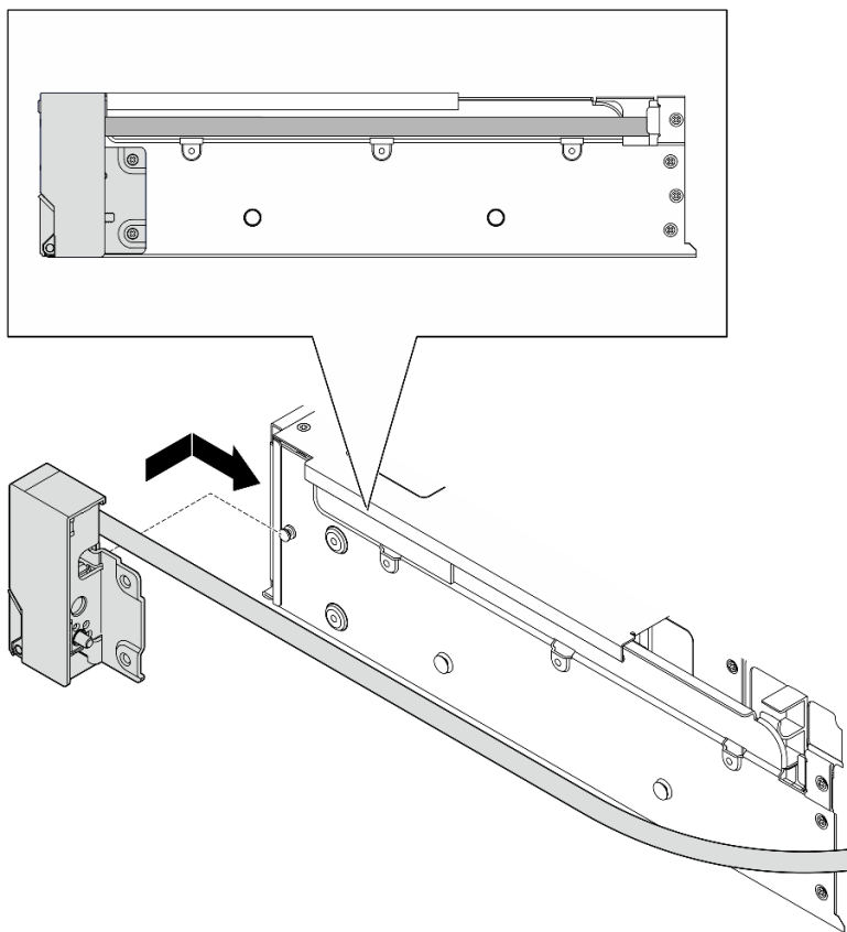
Figura 202. Instalando a trava do rack
