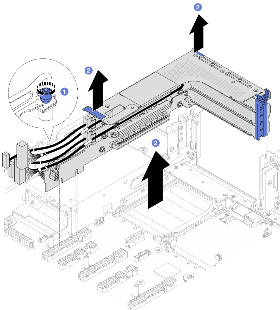
Figura 212. Remoção do conjunto de placa riser 3FH
