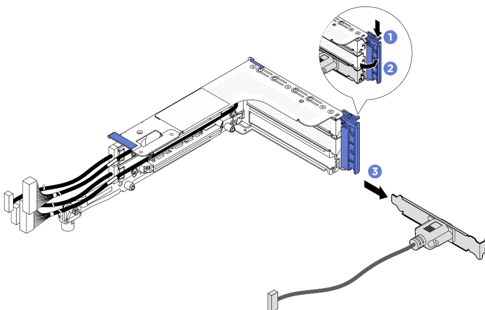
Figura 225. Removendo o módulo de porta serial
