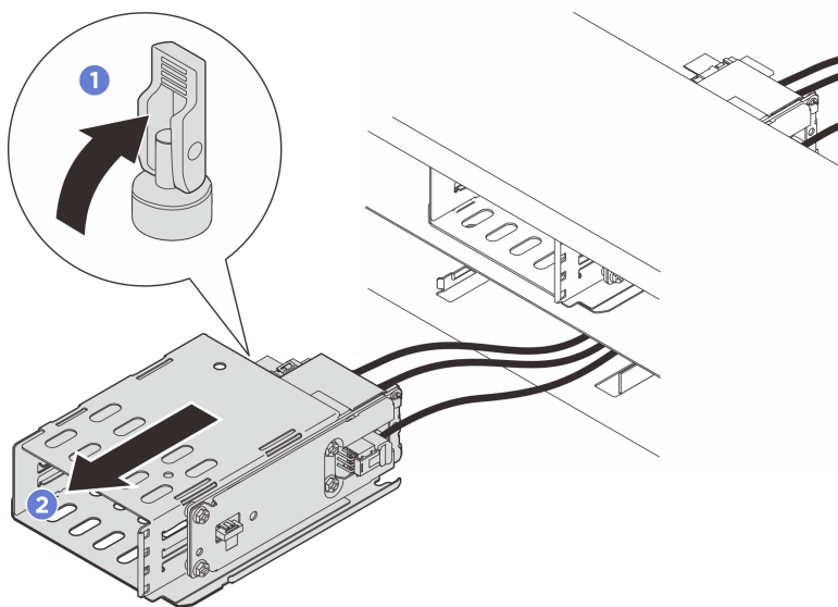
Figura 46. Remoção da gaiola E3.S 1T
