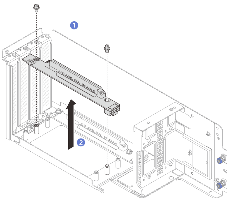
Figura 62. Remoção da placa riser
