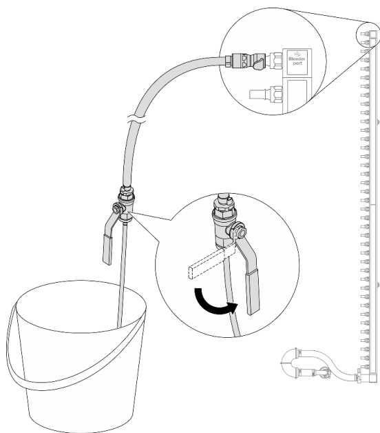
Figura 147. Abrindo a válvula de drenagem
