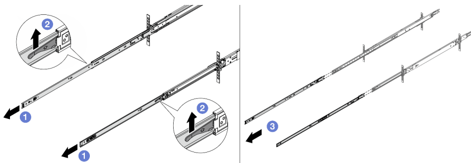
Figura 11. Puxando os trilhos
