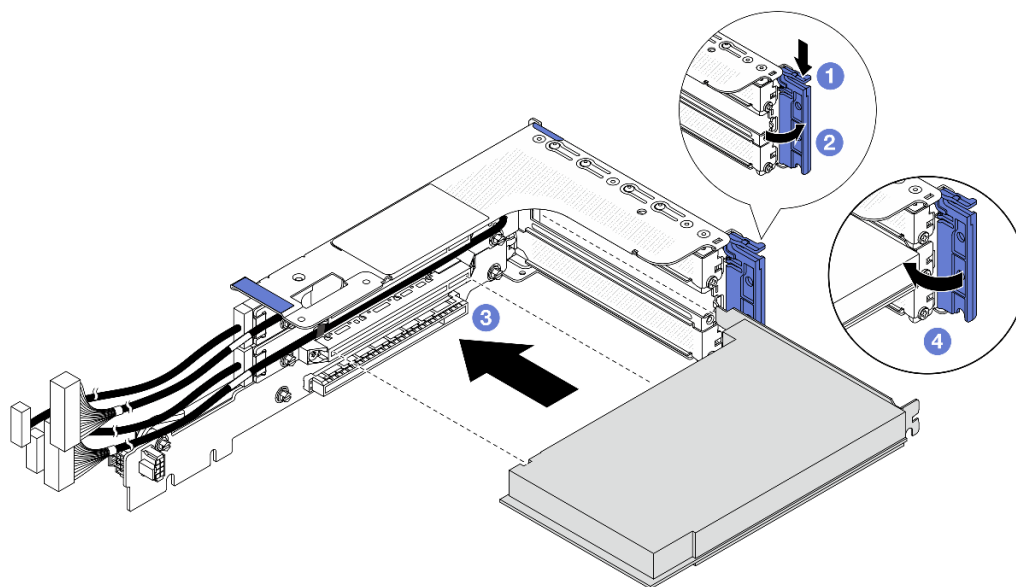
Figura 216. Instalação de um adaptador PCIe na gaiola da placa riser 3FH
