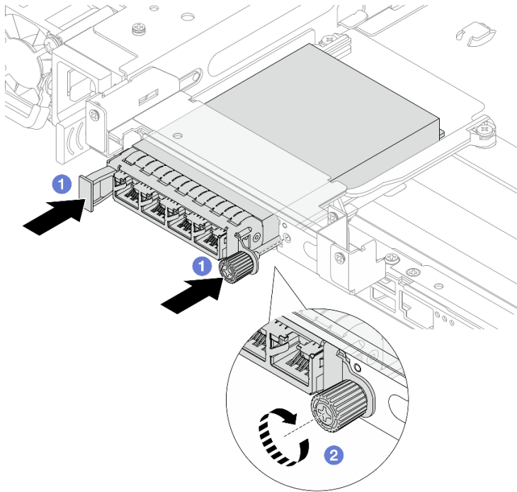
Figura 209. Instalando o módulo OCP traseiro
