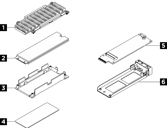
Figura 104. Partes de um conjunto de unidade M.2 hot-swap
