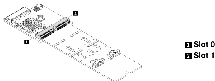
Figura 80. Slot da unidade M.2
