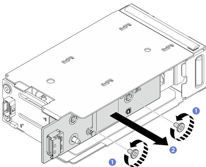
Figura 120. Remoção da placa do controlador M.2 frontal
