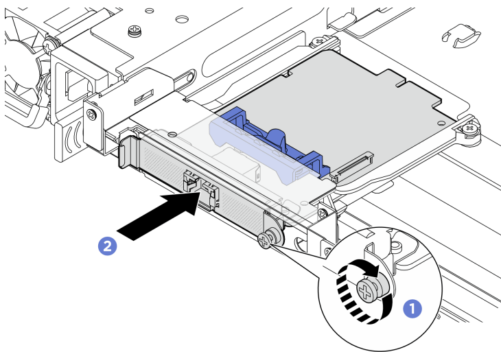
Figura 133. Instalando o adaptador NIC de gerenciamento
