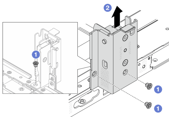
Figura 218. Remoção do suporte da parede traseira esquerda
