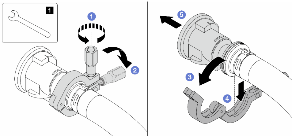
Figura 150. Separando válvulas esféricas
