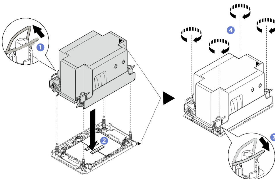
Figura 197. Instalação de um PHM padrão 2U
