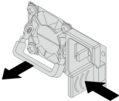
Figura 69. Remoção da unidade de fonte de alimentação hot-swap
