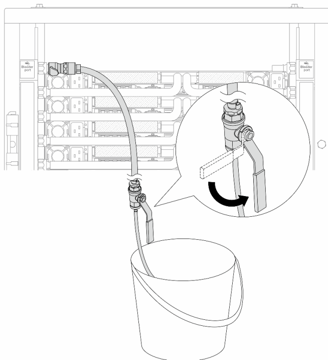
Figura 180. Abrindo a válvula de drenagem no lado de abastecimento
