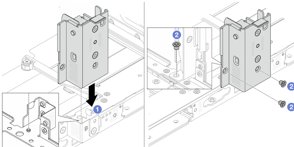
Figura 222. Instalação do suporte de parede traseira central
