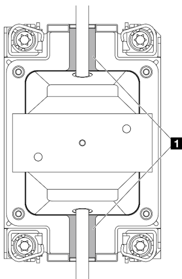
Figura 263. Áreas propensas a vazamentos
