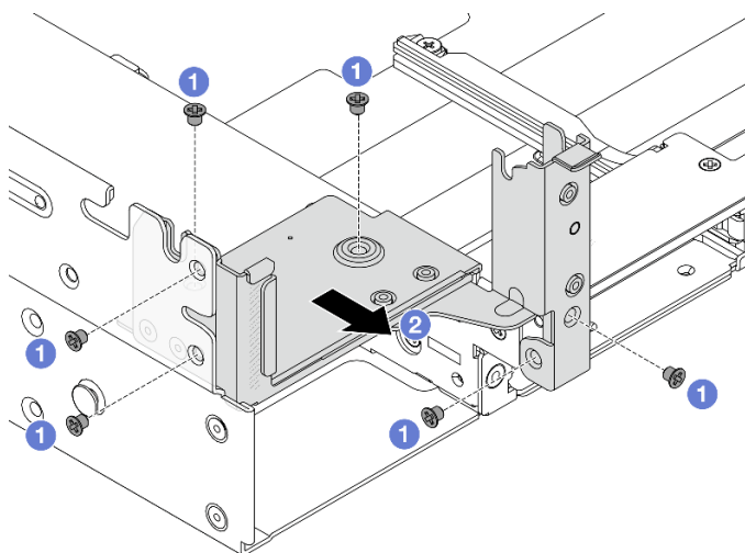
Figura 218. Remoção do suporte da parede traseira esquerda
