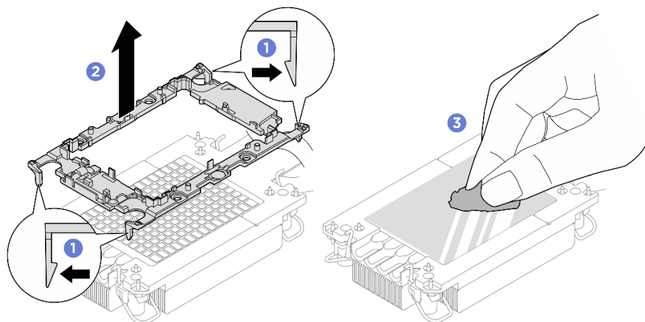
Figura 191. Separando a portadora do processador do dissipador de calor
