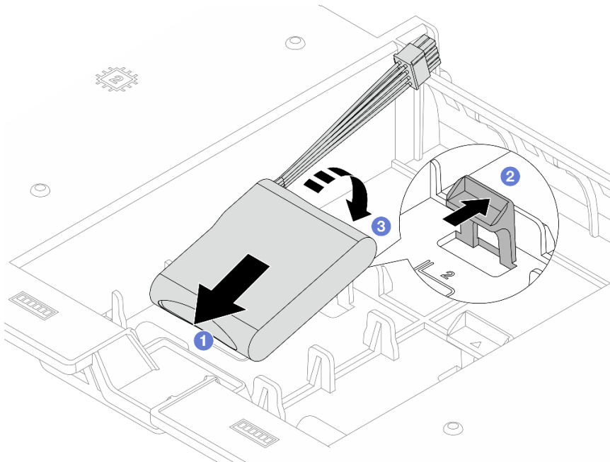
Figura 207. Instalando o módulo de energia flash RAID no defletor de ar
