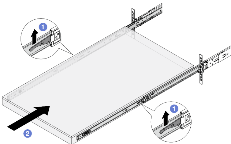
Figura 15. Travando os trilhos e deslizando no servidor
