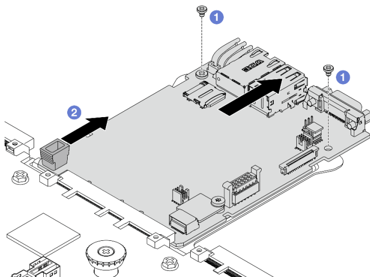
Figura 232. Separando a placa de E/S do sistema da placa do processador
