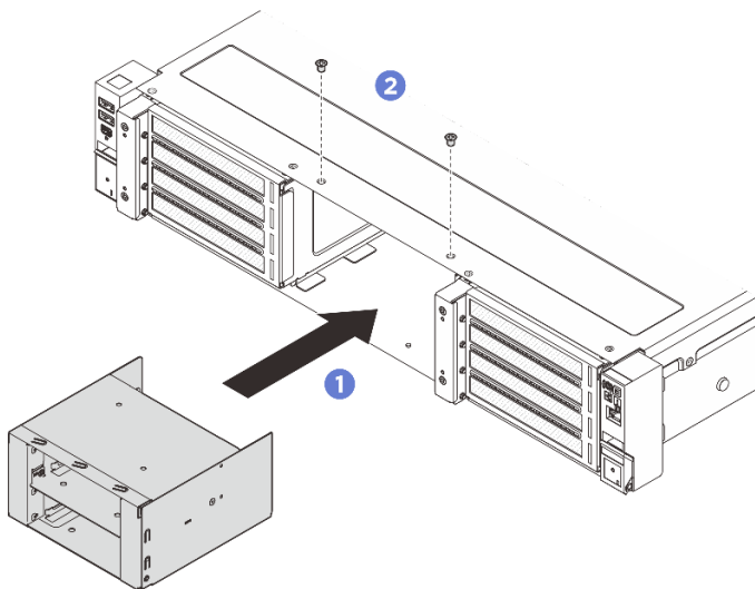
Figura 49. Instalação da gaiola E3.S
