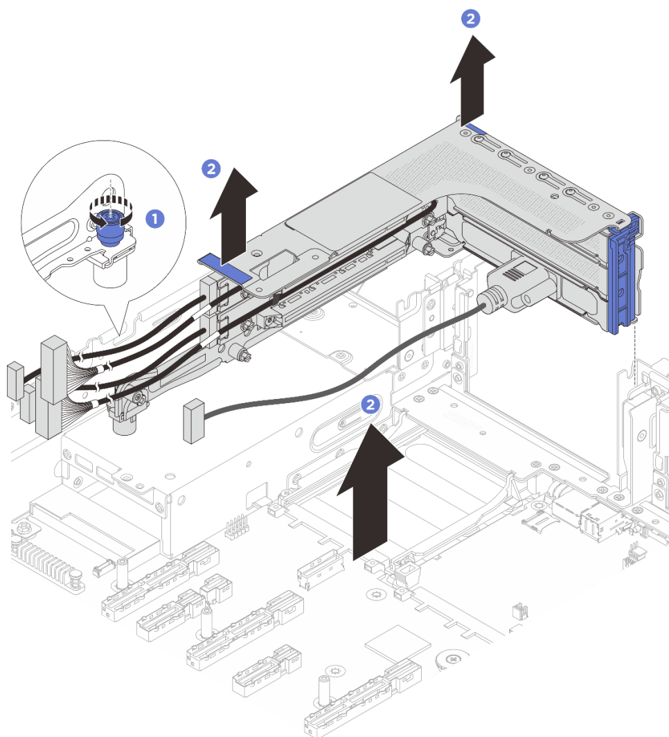
Figura 224. Removendo o conjunto de placa riser
