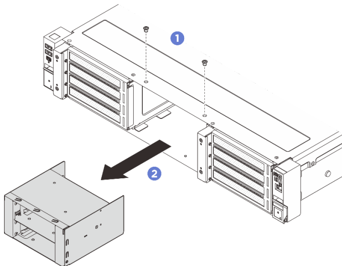
Figura 48. Remoção da gaiola de unidade E3.S
