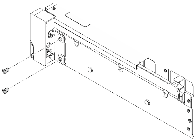
Figura 203. Instalando os parafusos
