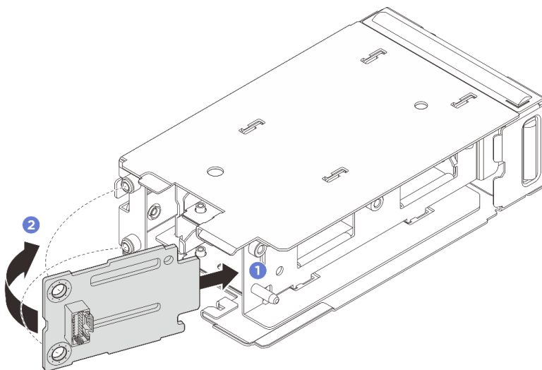
Figura 124. Instalação do backplane de inicialização M.2
