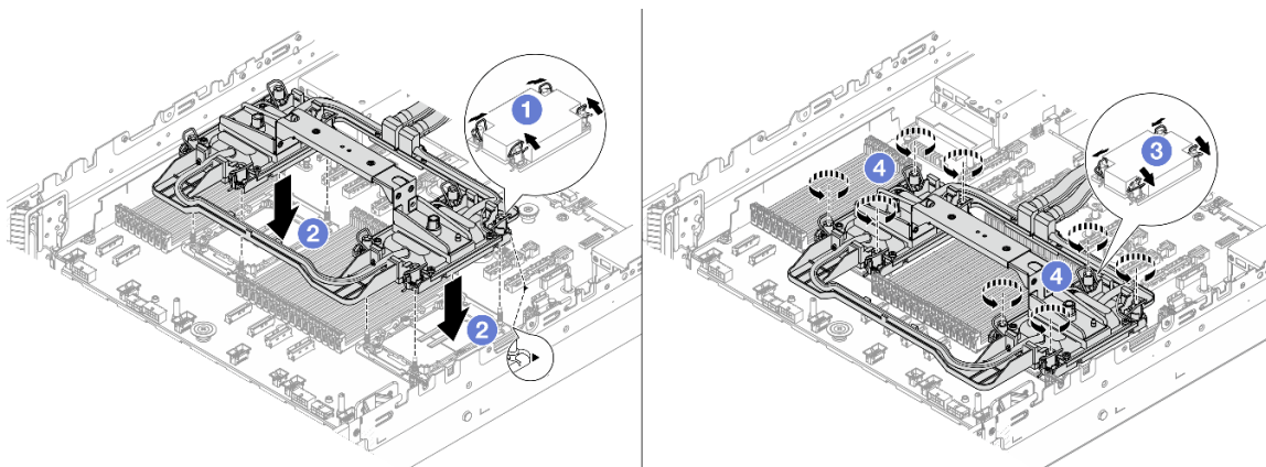
Figura 97. Instalando a Processor Neptune Core Module
