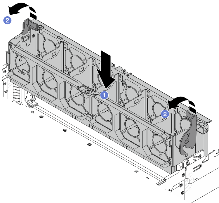
Figura 242. Instalando a gaiola do ventilador do sistema
