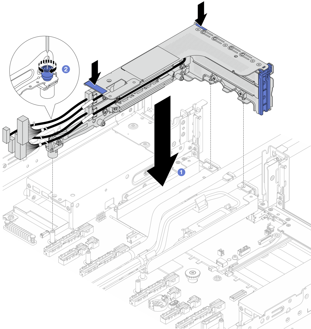
Figura 103. Instalando a gaiola de placa riser 3FH
