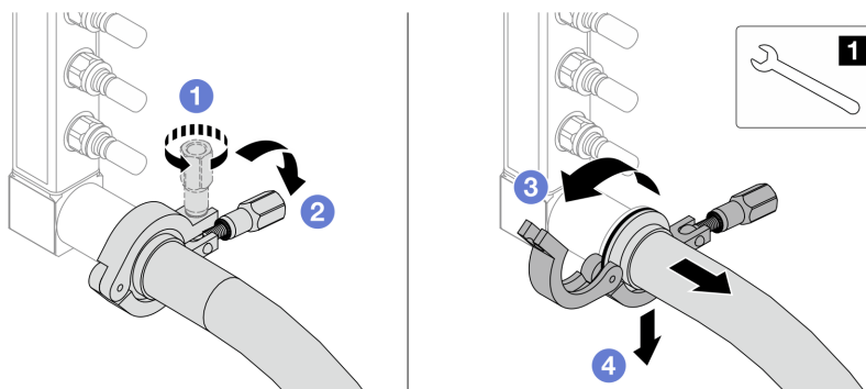
Figura 148. Separando o coletor do conjunto de conexões
