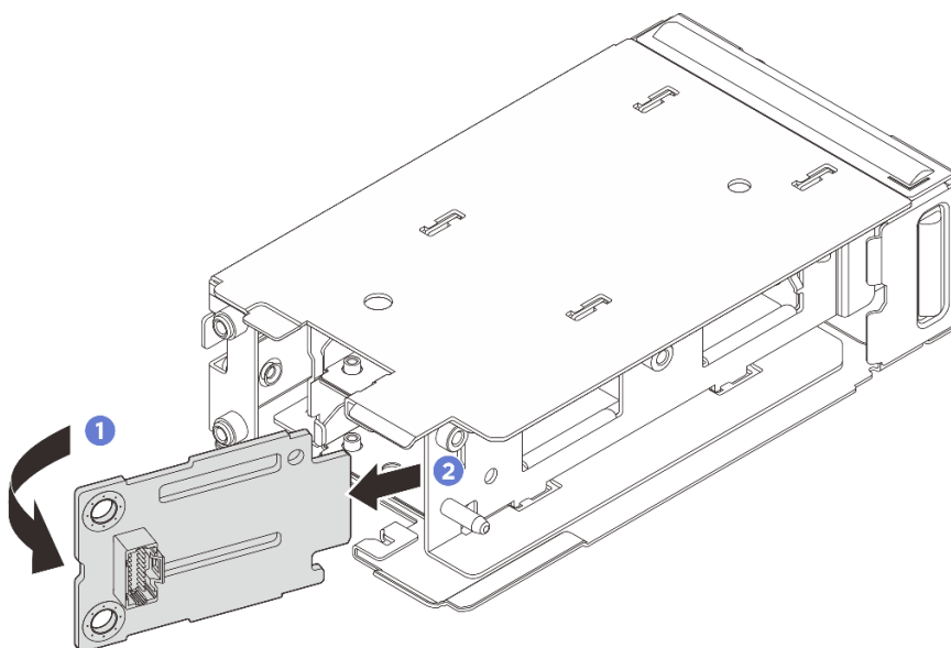
Figura 122. Remoção do backplane de inicialização M.2 frontal
