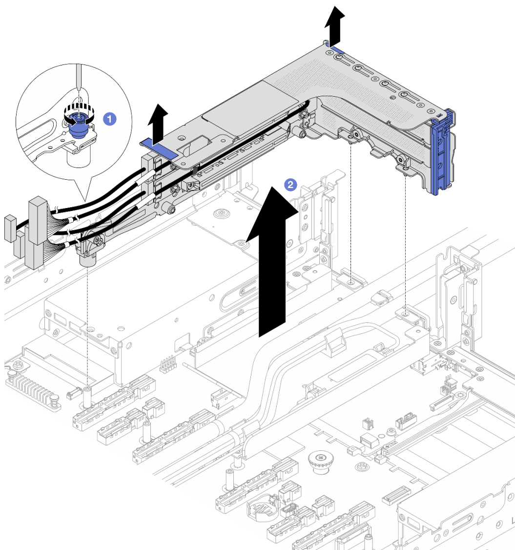
Figura 90. Removendo a gaiola de placa riser 3FH
