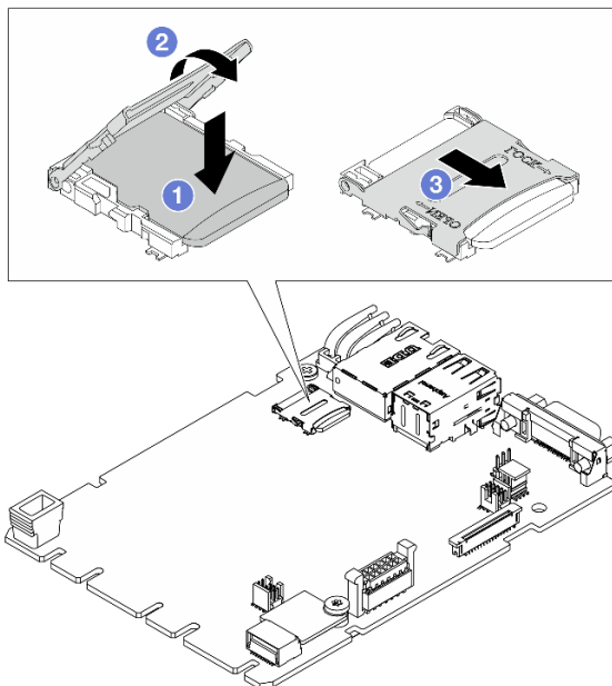
Figura 185. Instalando o cartão MicroSD
