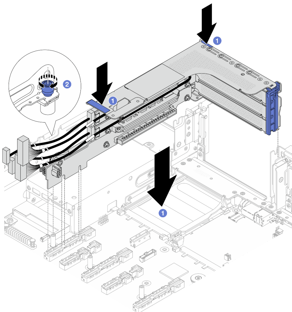
Figura 217. Instalação do conjunto de placa riser 3FH
