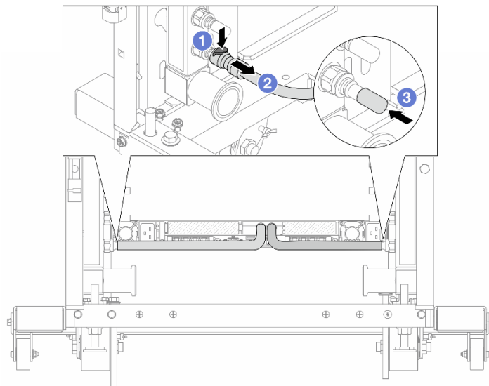
Figura 164. Remoção dos plugues de conexão rápida
