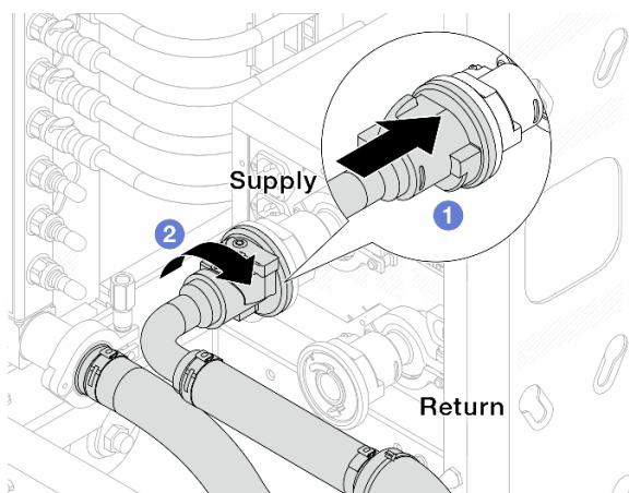
Figura 153. Conectando válvulas esféricas
