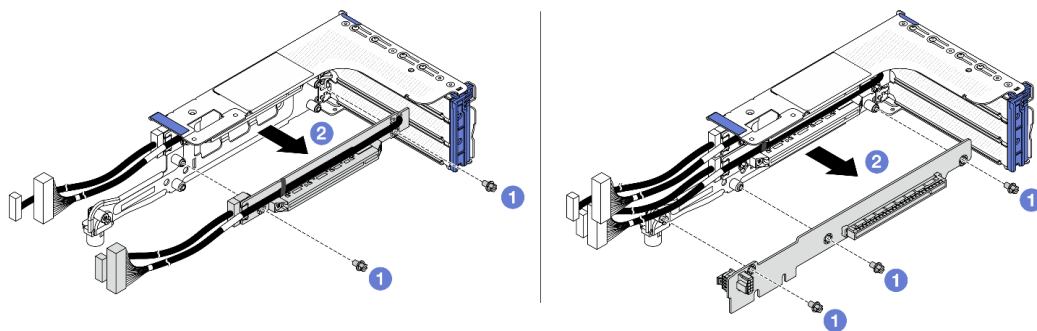
Figura 214. Remoção de placas riser da gaiola
