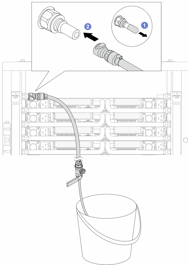
Figura 157. Instalando o kit de drenagem no lado de abastecimento
