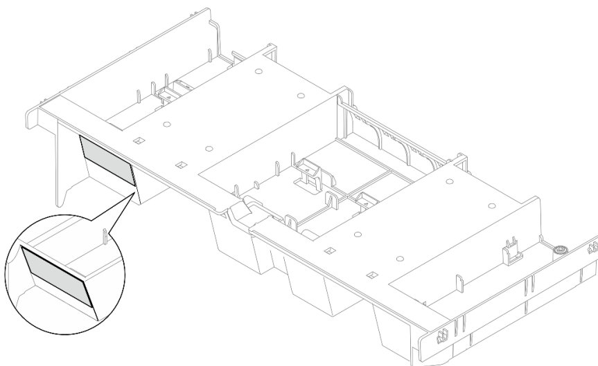
Figura 30. Mylar do defletor de ar
