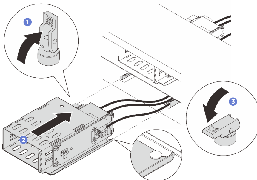
Figura 51. Instalação da gaiola E3.S 1T
