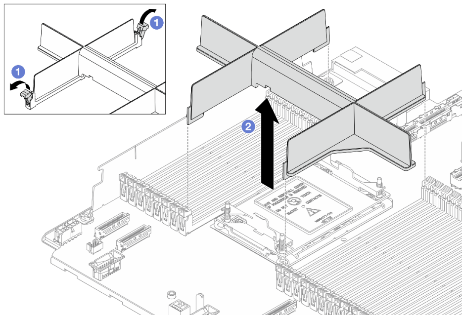
Figura 196. Removendo um preenchimento PHM
