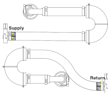
Figura 138. Conjunto de conexões em rack 42U
