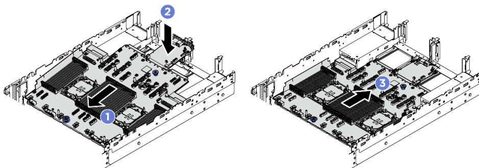
Figura 234. Instalando o conjunto de placa-mãe
