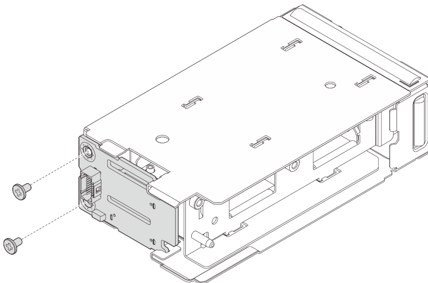
Figura 121. Remoção do backplane de inicialização M.2 frontal
