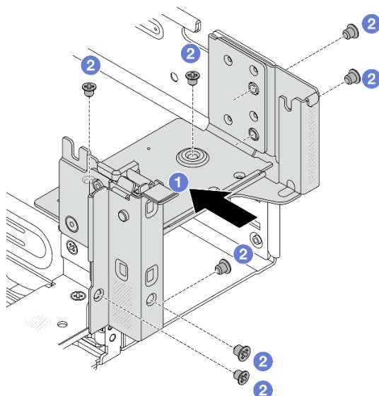
Figura 223. Instalando o suporte de parede traseira direito
