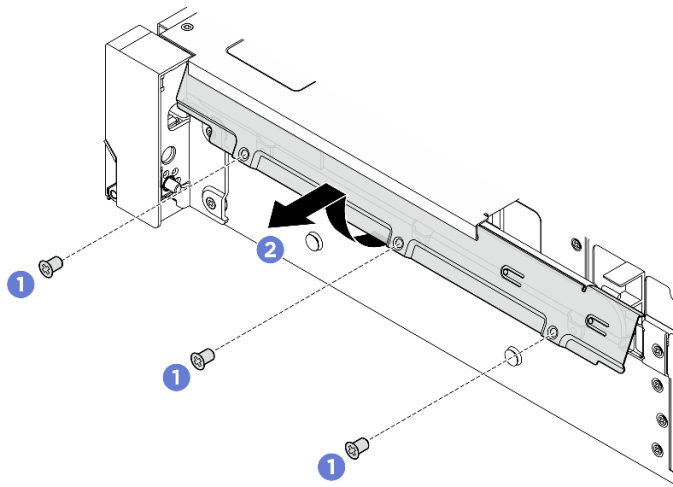
Figura 199. Removendo o retentor de cabo
