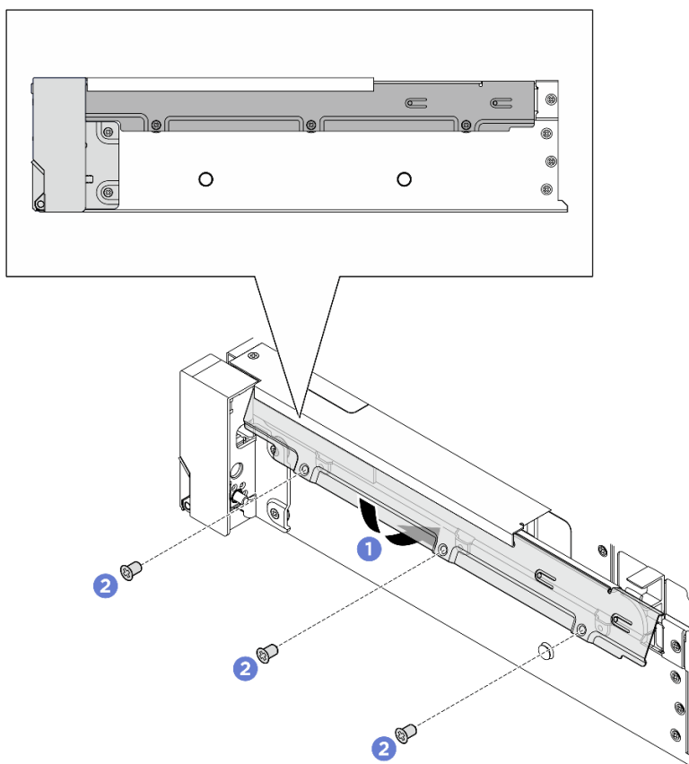
Figura 204. Instalando o retentor de cabos
