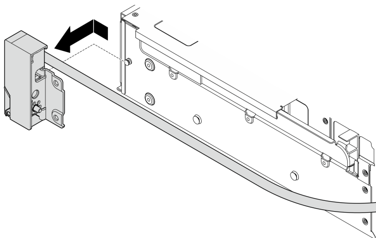
Figura 201. Removendo a trava do rack
