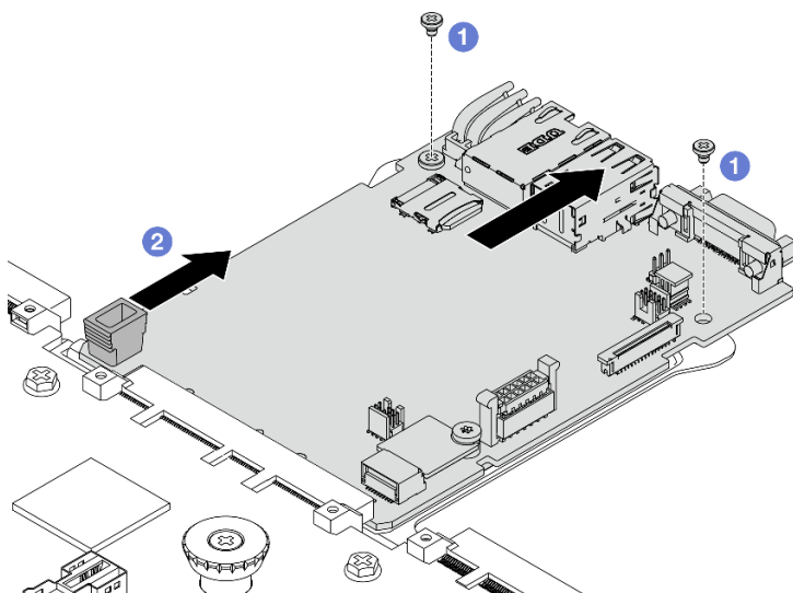
Figura 236. Separando a placa de E/S do sistema da placa do processador
