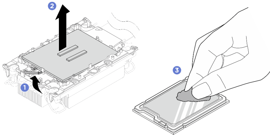
Figura 190. Separando o processador do dissipador de calor e da portadora
