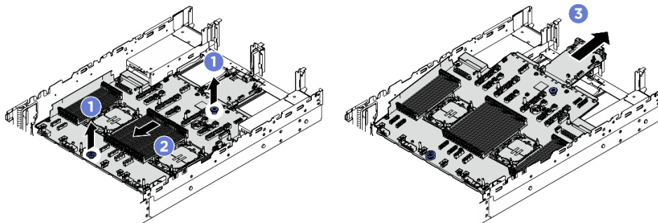
Figura 231. Removendo o conjunto de placa-mãe
