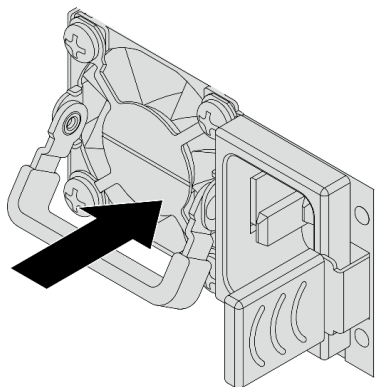
Figura 73. Instalação da unidade da fonte de alimentação hot-swap
