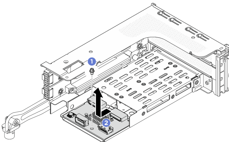
Figura 130. Remoção do backplane M.2 da gaiola da placa riser 3FH M.2
