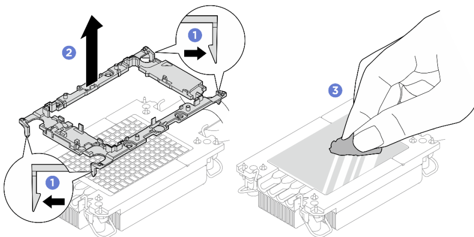
Рис. 191. Снятие держателя процессора с радиатора
