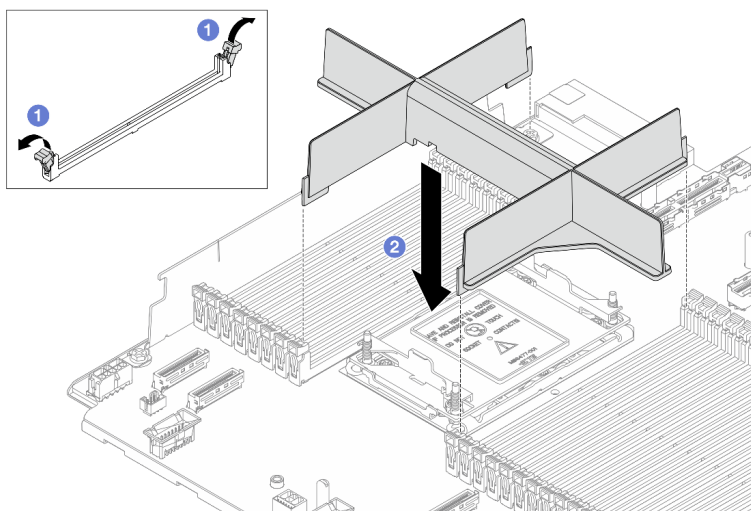
Рис. 189. Установка заглушки РНМ
