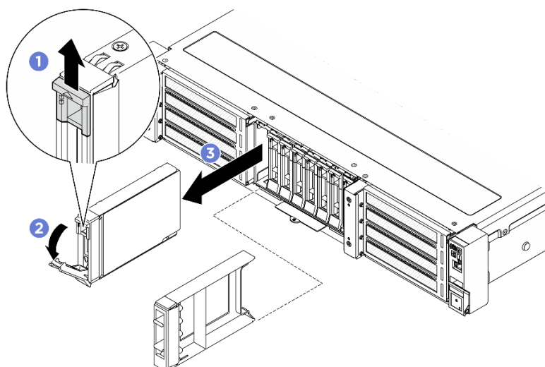
Рис. 18. Снятие 2,5-дюймового оперативно заменяемого диска
