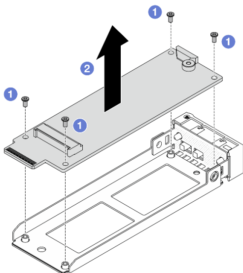
Рис. 110. Снятие интерпозера M.2
