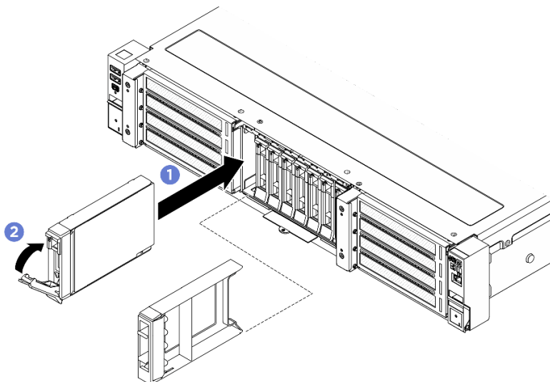
Рис. 20. Установка 2,5-дюймового оперативно заменяемого диска
