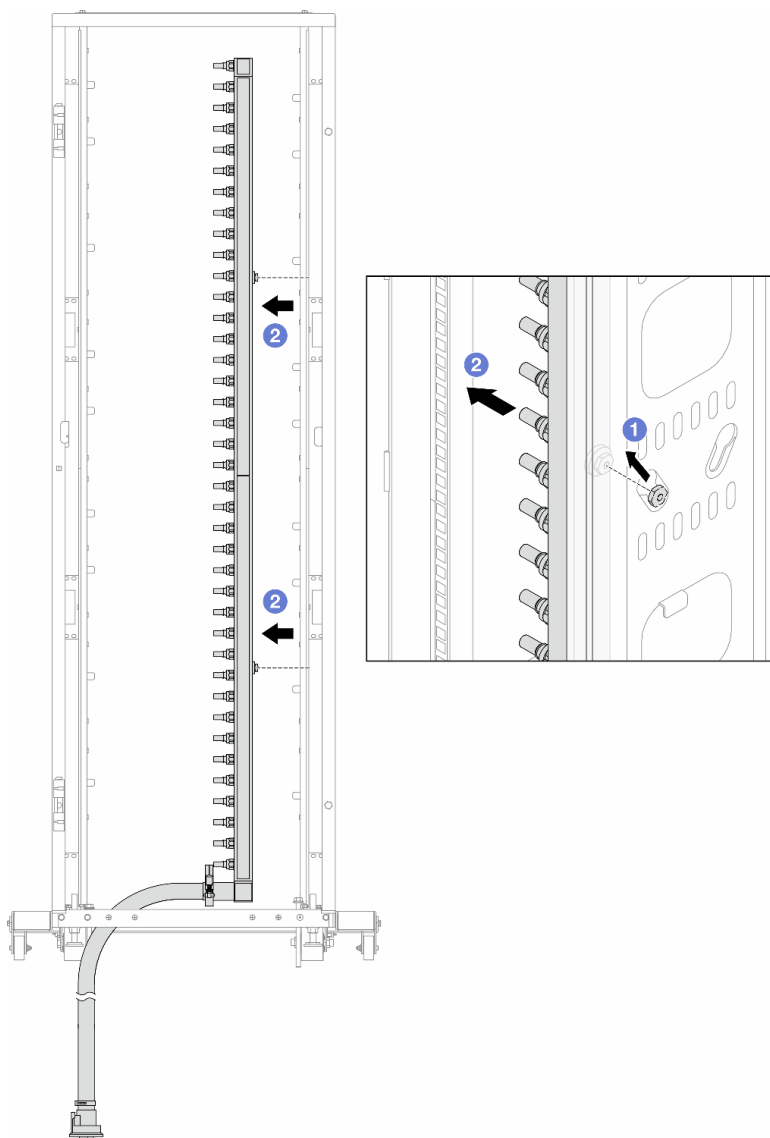
Рис. 165. Снятие коллектора
