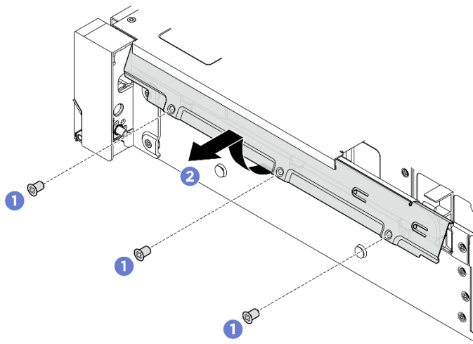
Рис. 199. Снятие фиксатора кабелей
