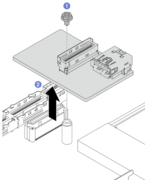
Рис. 246. Снятие платы ввода-вывода USB
