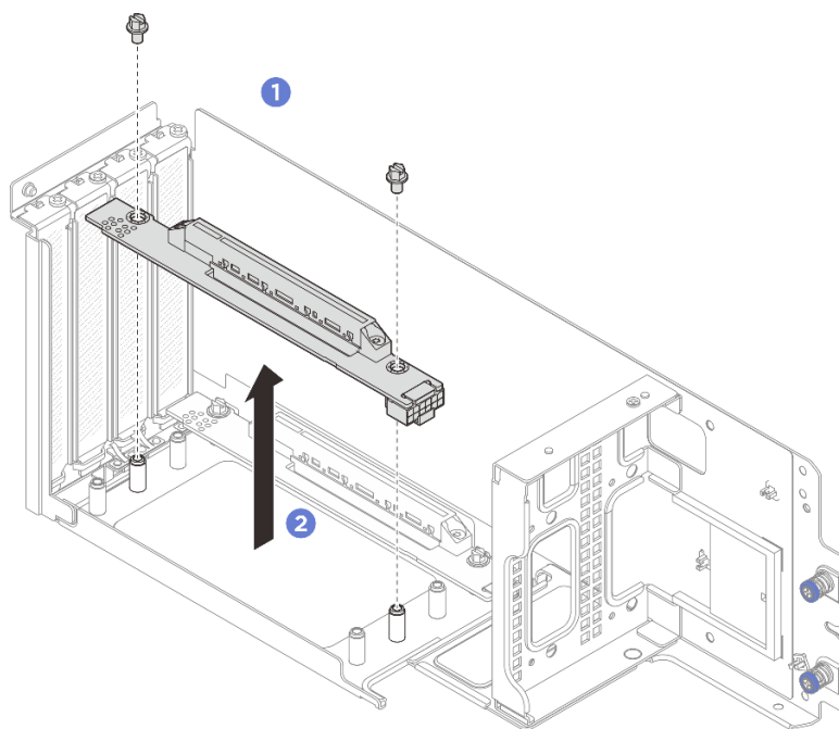
Рис. 62. Снятие платы-адаптера Riser
