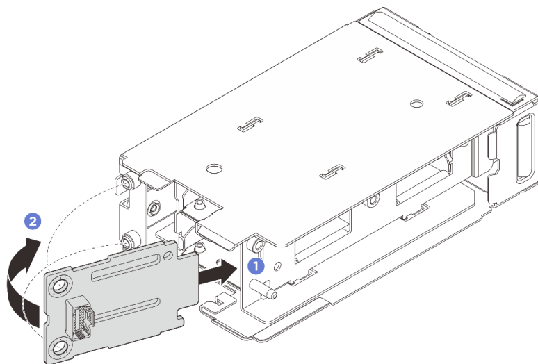
Рис. 124. Установка объединительной панели загрузки M.2
