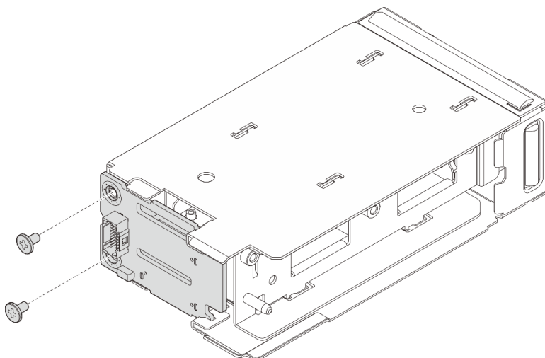
Рис. 125. Установка объединительной панели загрузки M.2
