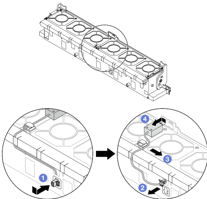
Рис. 87. Снятие датчика вмешательства
