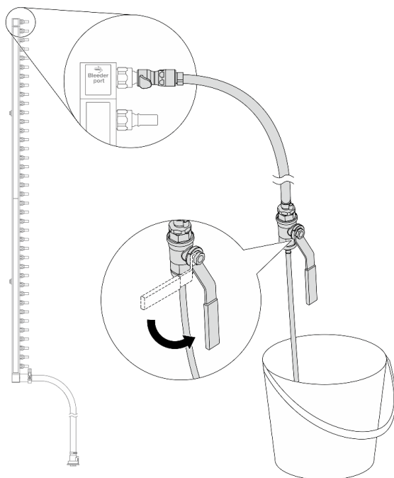
Рис. 167. Открытие клапана отводной трубки
