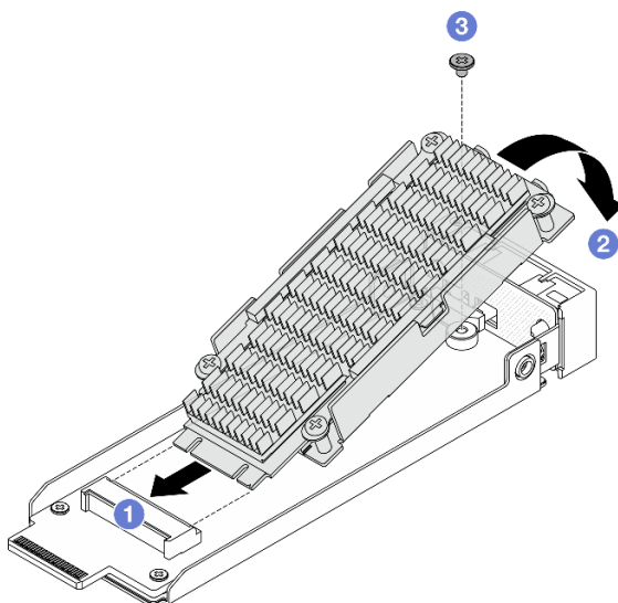
Рис. 116. Установка диска M.2 с радиатором
