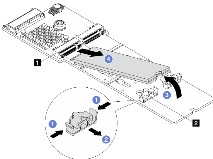
Рис. 78. Снятие диска M.2
