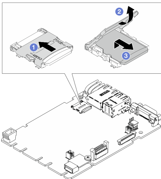
Рис. 184. Извлечение карты microSD
