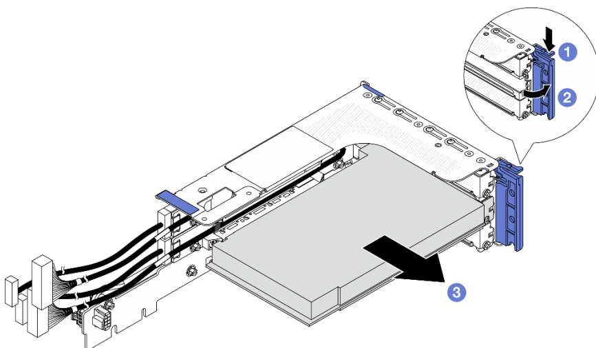
Рис. 213. Снятие адаптера PCIe с отсека платы-адаптера Riser 3FH
