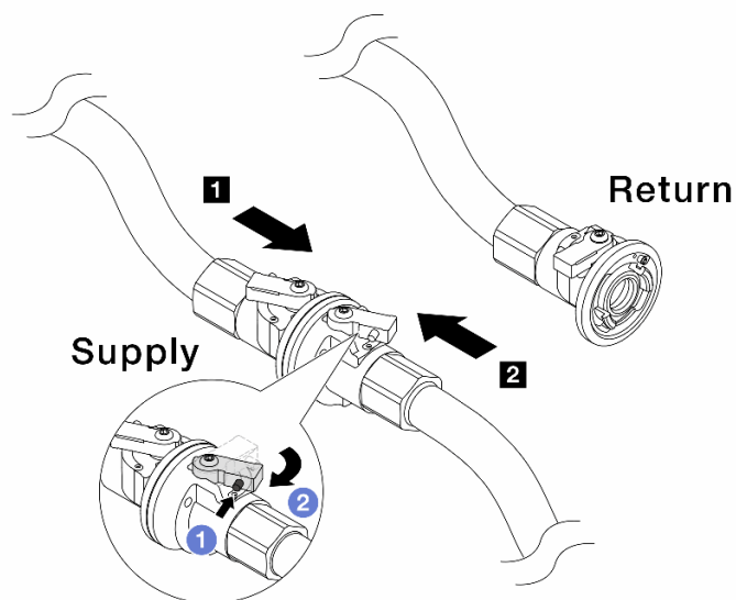
Рис. 178. Подключение разъема на стороне подачи объекта к разъему на стороне подачи коллектора
