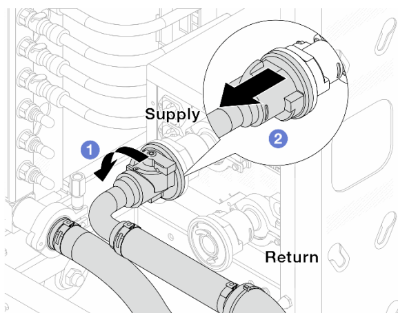
Рис. 142. Снятие комплекта соединений
