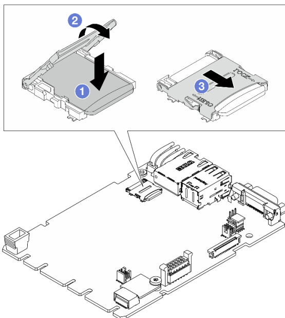
Рис. 185. Установка карты MicroSD
