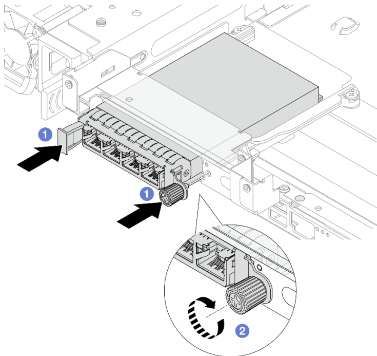
Рис. 209. Установка заднего модуля ОСР
