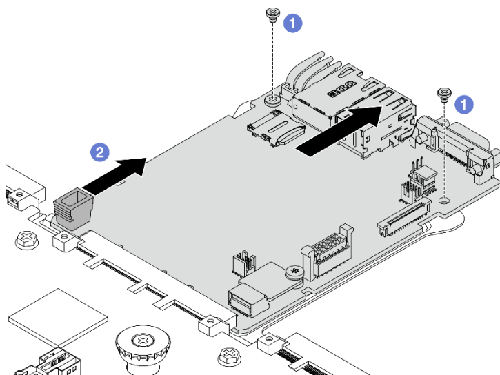
Рис. 232. Снятие системной платы ввода-вывода с процессорной платы
