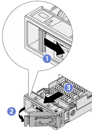
Рис. 105. Снятие блока оперативно заменяемых дисков M.2
