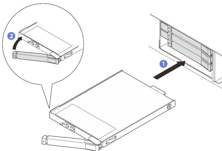
Рис. 41. Установка оперативно заменяемого диска E3.S
