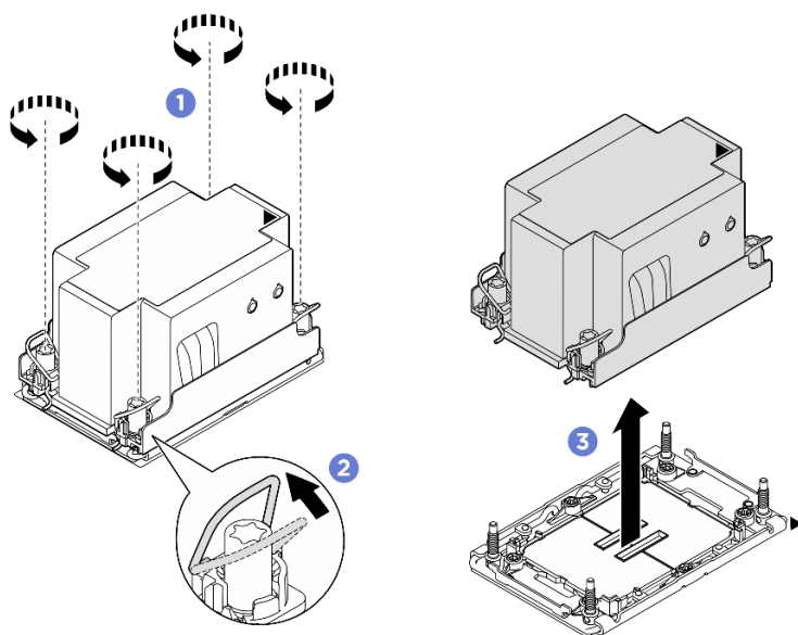
Рис. 187. Снятие стандартного модуля PNM 2U
