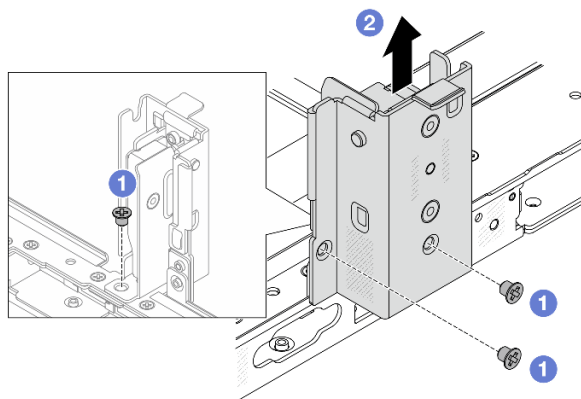
Рис. 218. Снятие левой скобы задней стенки
