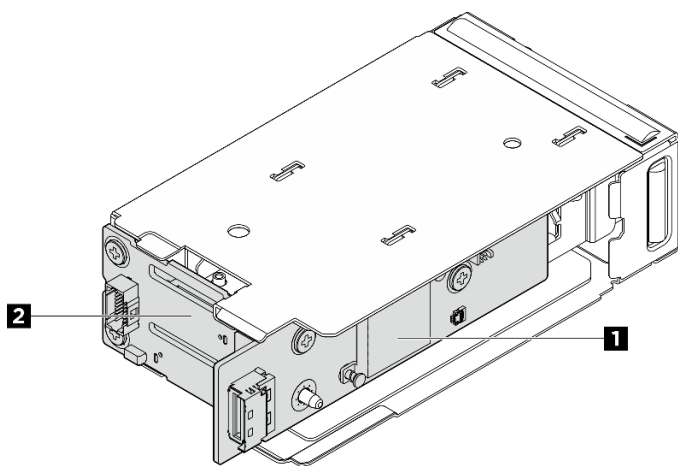
Рис. 123. Передние объединительные панели для дисков M.2
