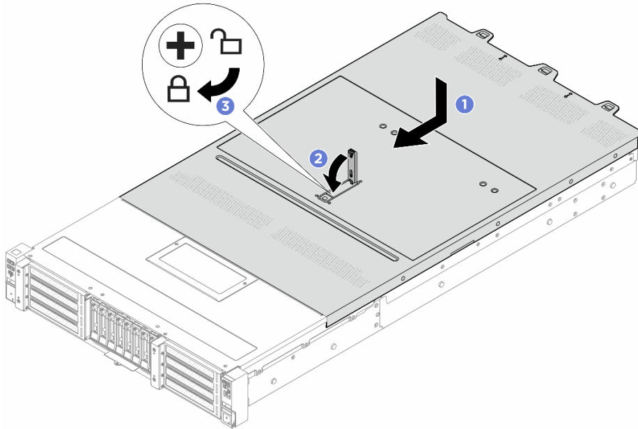
Рис. 245. Установка верхнего кожуха
