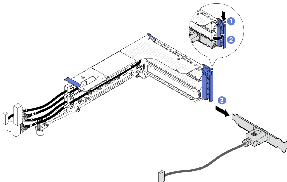
Рис. 225. Извлечение модуля последовательного порта
