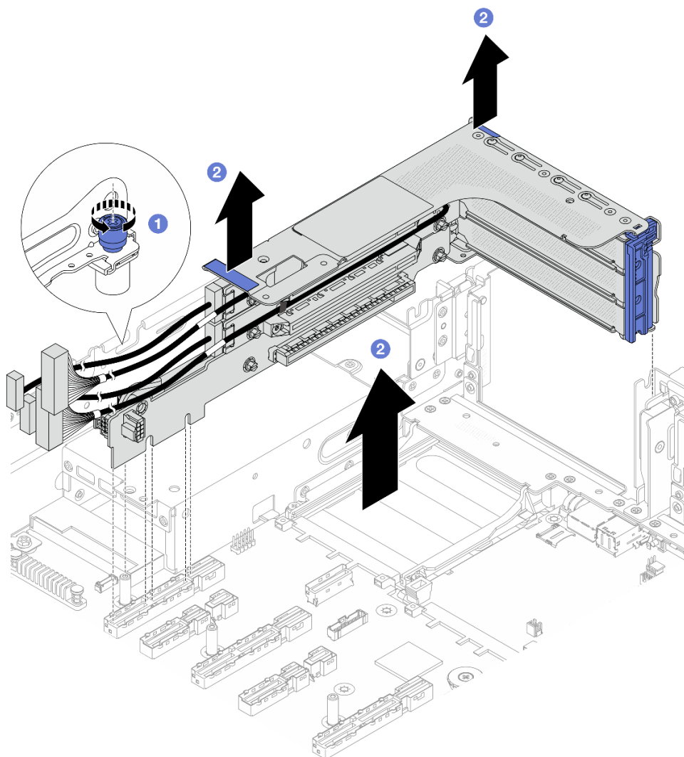
Рис. 212. Снятие блока платы-адаптера Riser 3FH
