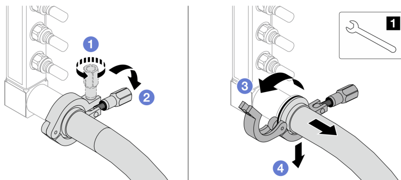
Рис. 170. Отделение коллектора от комплекта шланга
