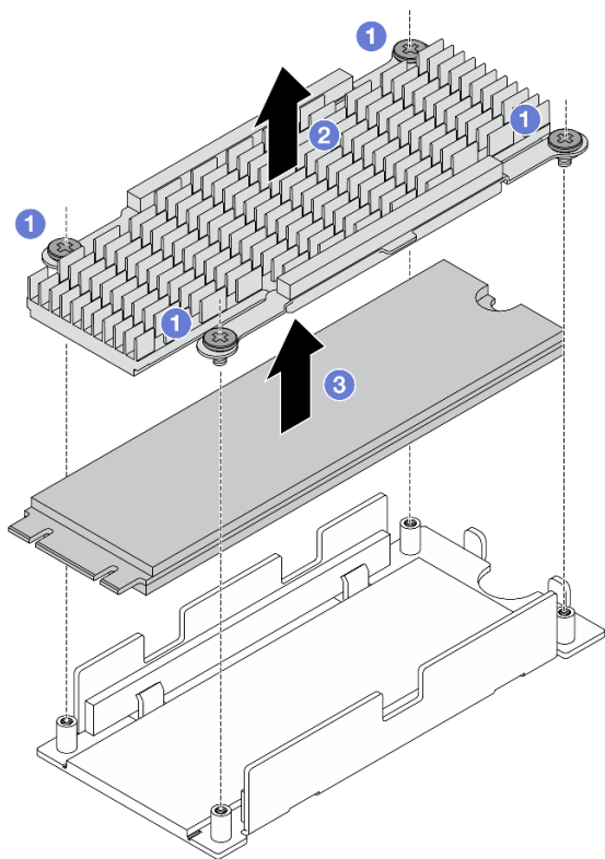
Рис. 111. Снятие диска M.2
