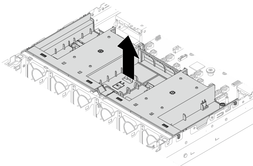
Рис. 27. Снятие дефлектора
