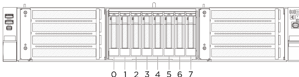
Рис. 19. Нумерация отсеков для 2,5-дюймовых дисков
