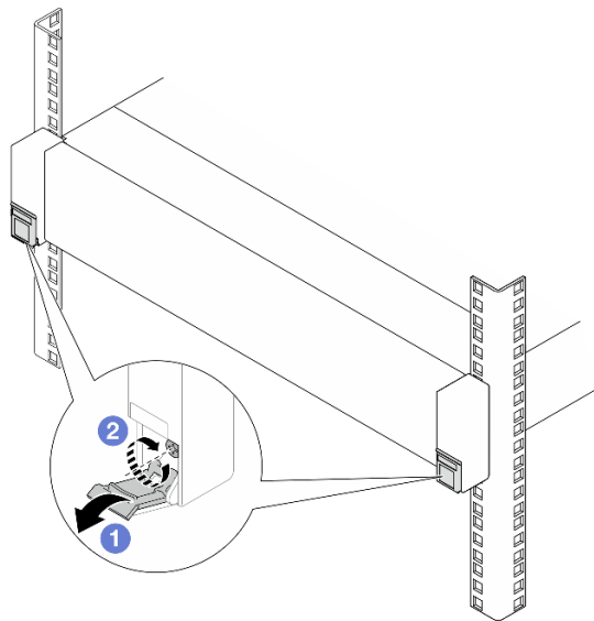
Рис. 16. Фиксация сервера на лицевой стороне стойки
