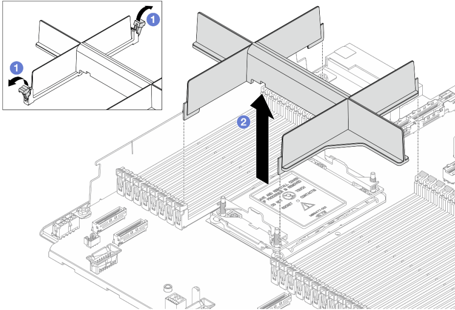
Рис. 196. Снятие заглушки РНМ
