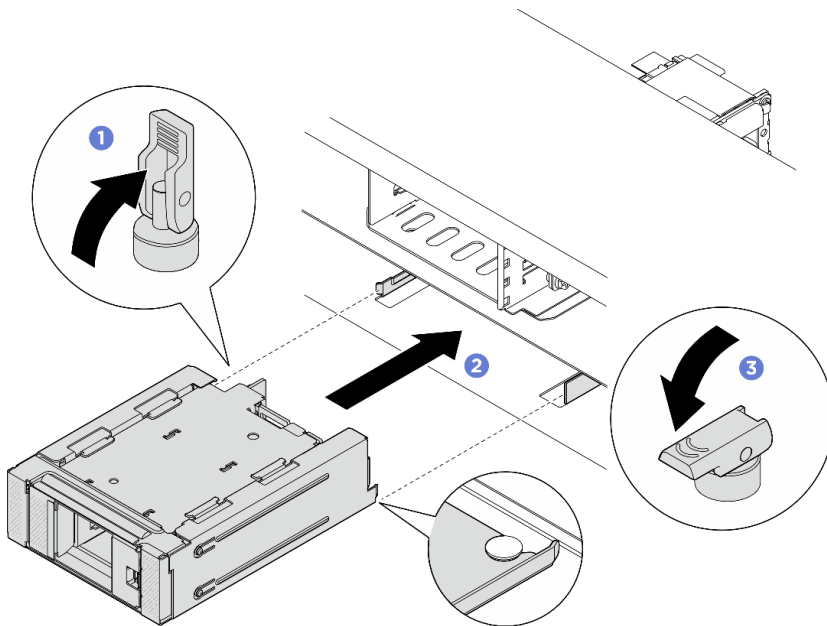
Рис. 128. Установка переднего отсека для дисков M.2 с корпусом
