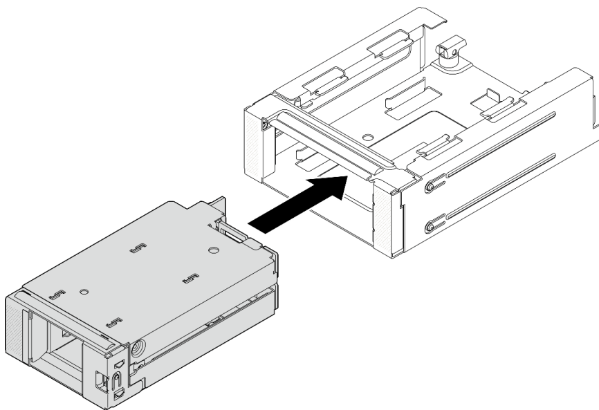
Рис. 127. Установка переднего отсека для дисков M.2 в корпус отсека
