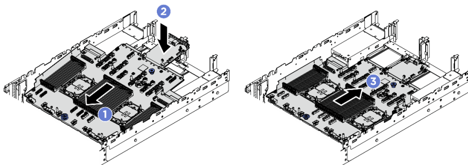
Рис. 238. Установка блока материнской платы
