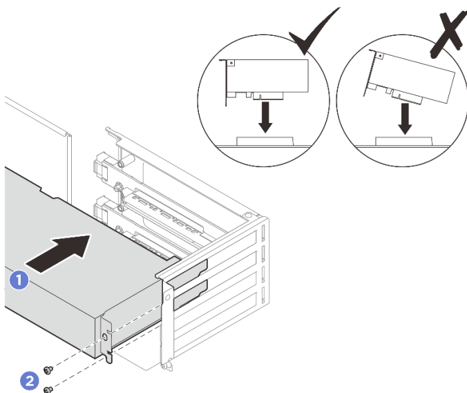
Рис. 57. Установка адаптера PCIe
