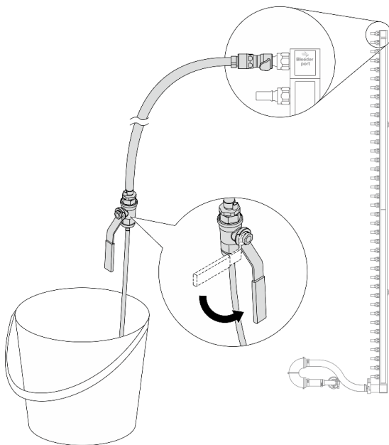
Рис. 147. Открытие клапана отводной трубы
