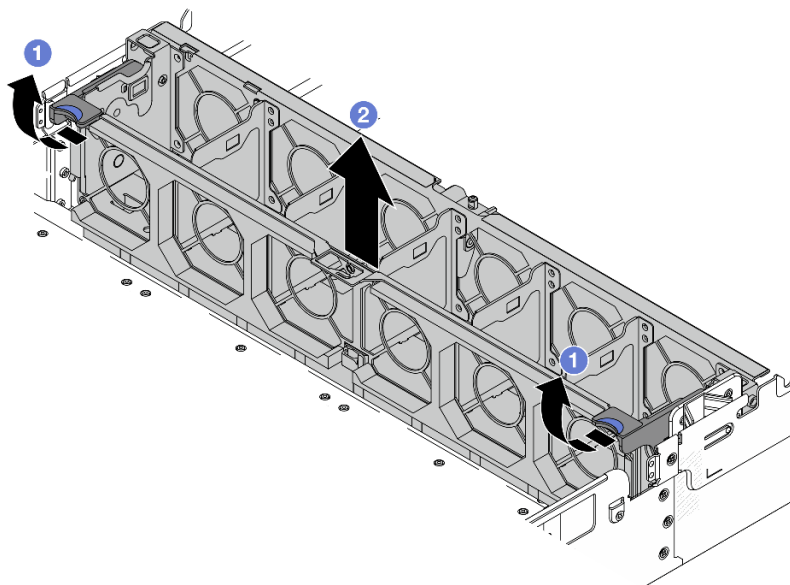
Рис. 241. Снятие отсека вентиляторов компьютера
