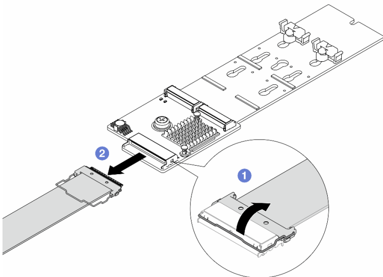
Рис. 82. Отключение кабеля M.2
