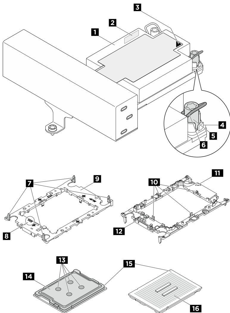
Рис. 192. Компоненты PNM
