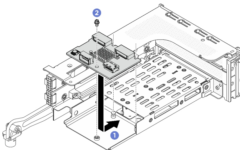
Рис. 131. Установка объединительной панели M.2 в отсек платы-адаптера Riser 3FH M.2
