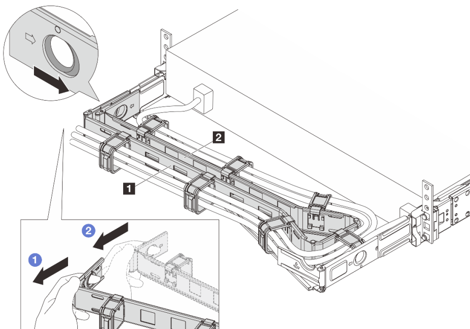
Рис. 68. Снятие левой стороны
