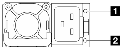
Рис. 258. Светодиодные индикаторы на модуле блока питания CRPS Premium
