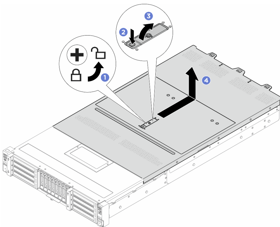
Рис. 243. Снятие верхнего кожуха
