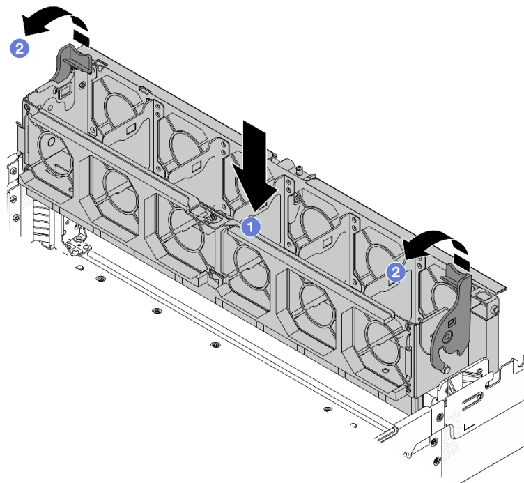
Рис. 242. Установка отсека вентиляторов компьютера
