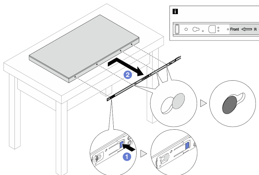
Рис. 10. Снятие внутренних направляющих
