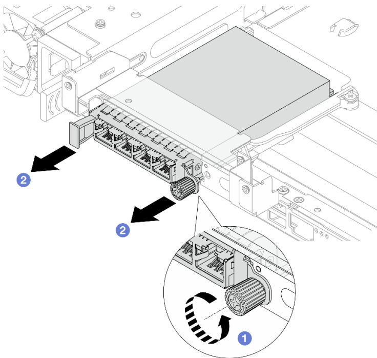
Рис. 208. Снятие заднего модуля ОСР
