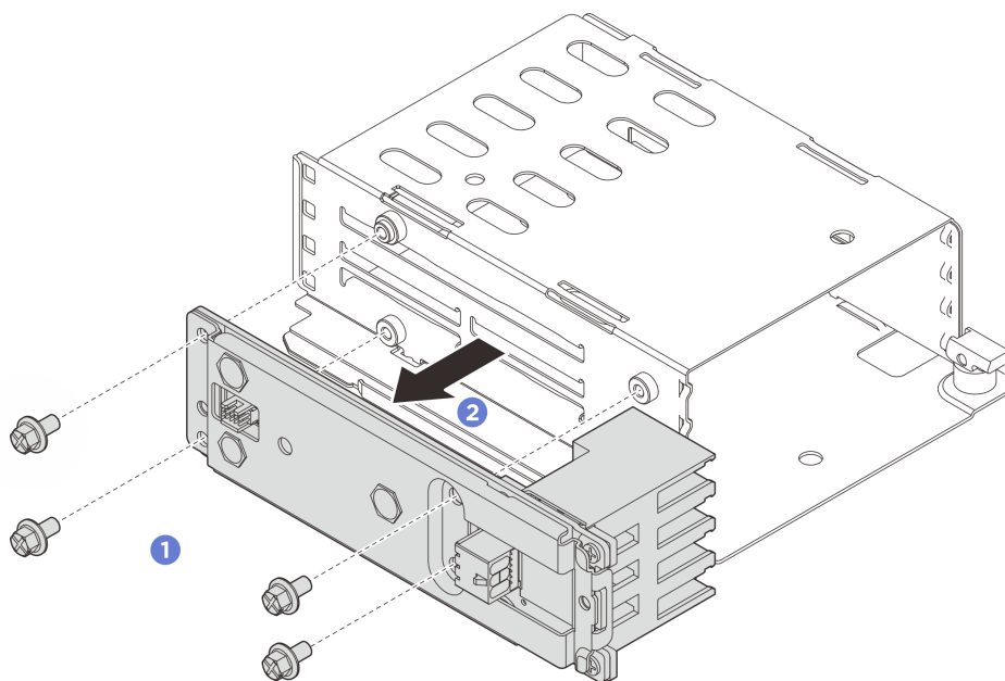
Рис. 47. Снятие блока объединительной панели
