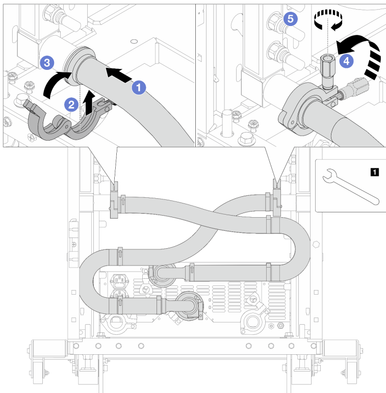
Рис. 152. Установка комплекта соединений
