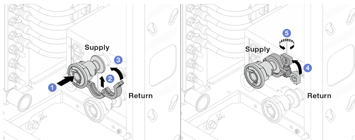
Рис. 151. Установка шаровых клапанов
