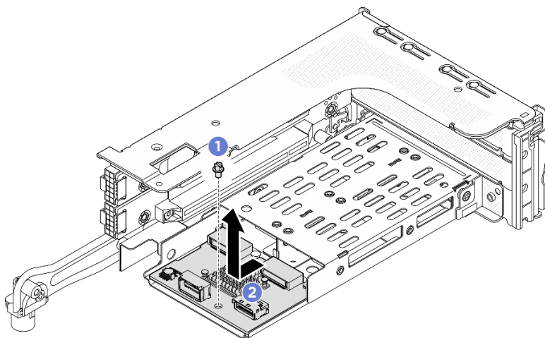
Рис. 130. Снятие объединительной панели M.2 с отсека платы-адаптера Riser 3FH M.2
