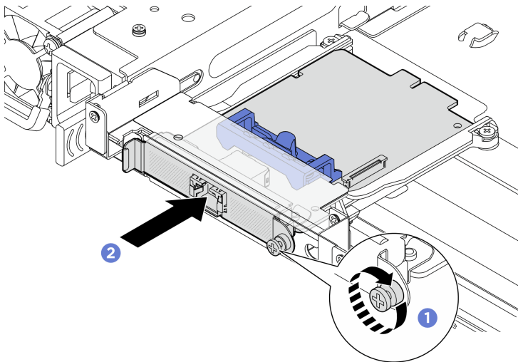
Рис. 133. Установка адаптера NIC для управления
