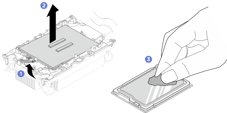
Рис. 190. Отделение процессора от радиатора и держателя
