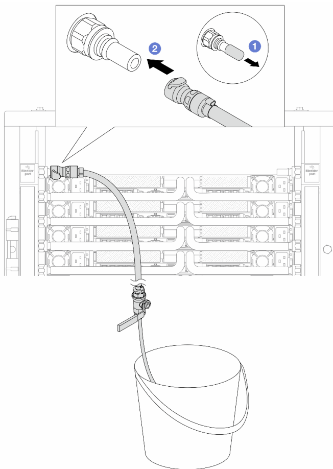
Рис. 174. Установка комплекта отводной трубки на стороне подачи
