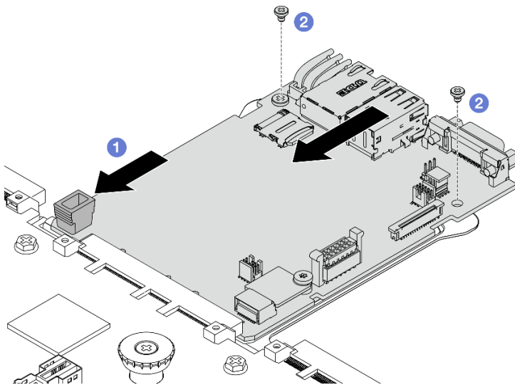
Рис. 233. Установка системной платы ввода-вывода на процессорную плату
