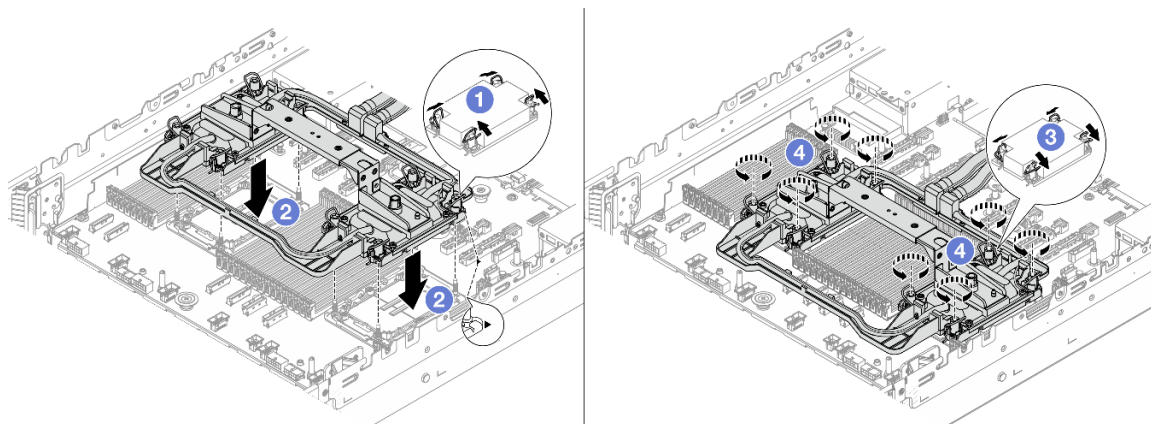
Рис. 97. Установка Processor Neptune Core Module
