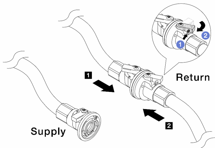
Рис. 175. Подключение разъема на стороне подачи объекта к разъему на стороне возврата коллектора
