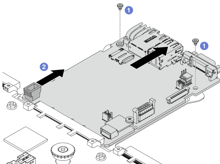
Рис. 236. Снятие системной платы ввода-вывода с процессорной платы
