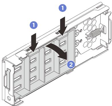
Рис. 43. Снятие внутренней пластины
