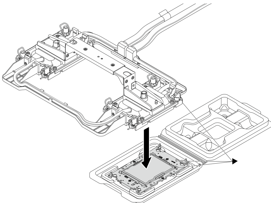
Рис. 95. Установка процессора
