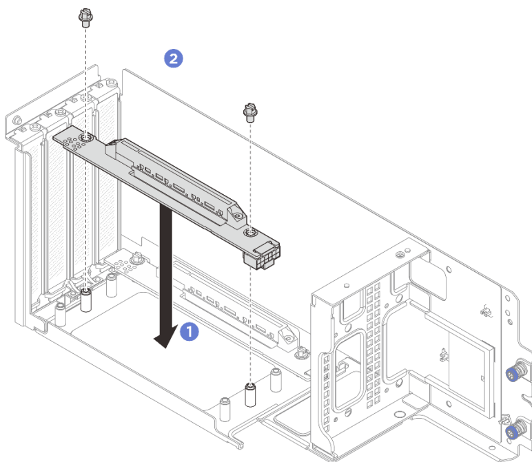
Рис. 63. Установка платы-адаптера Riser
