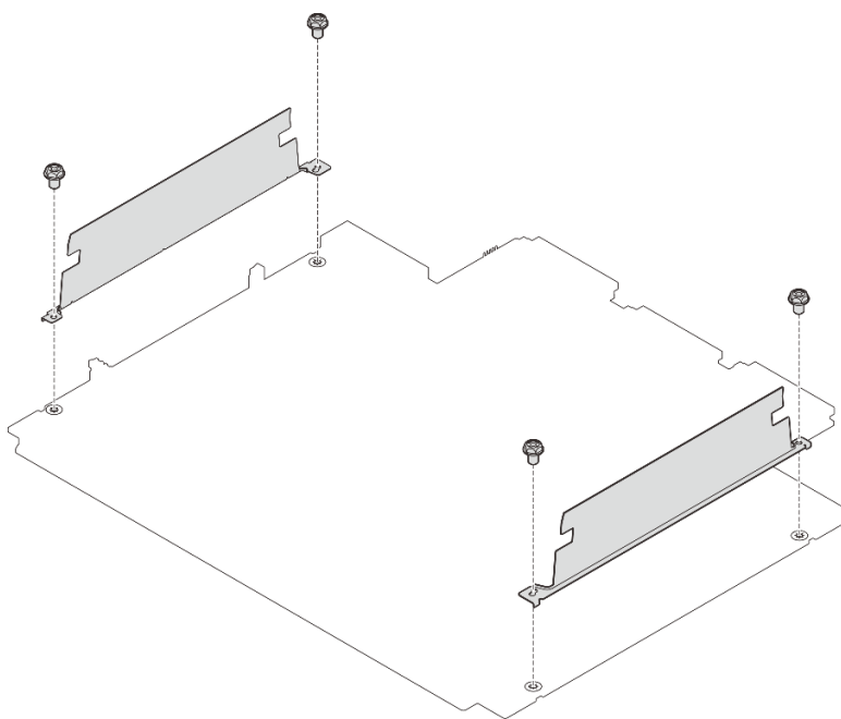
Рис. 33. Снятие стенок для кабелей
