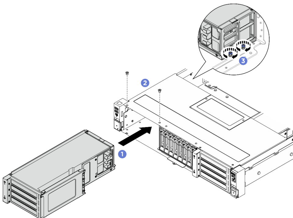
Рис. 60. Установка переднего блока платы-адаптера Riser
