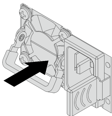
Рис. 73. Установка оперативно заменяемого модуля блока питания
