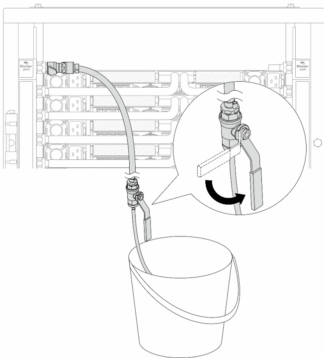
Рис. 159. Открытие клапана отводной трубки на стороне подачи
