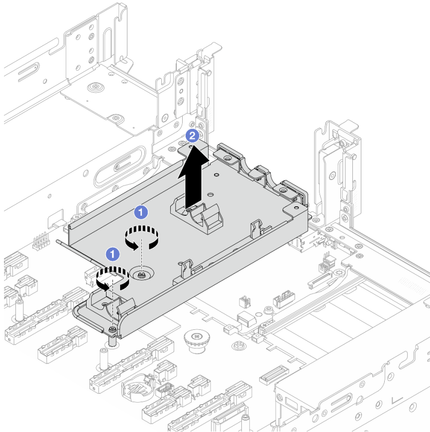
Рис. 93. Снятие держателя шланга
