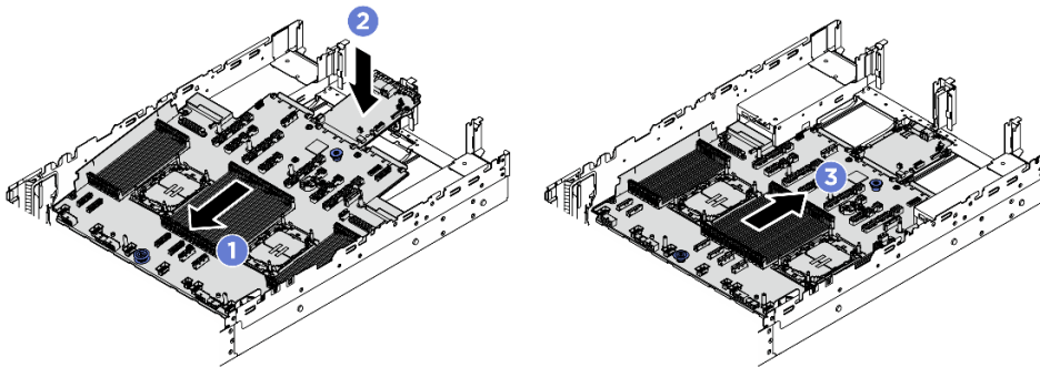
Рис. 234. Установка блока материнской платы
