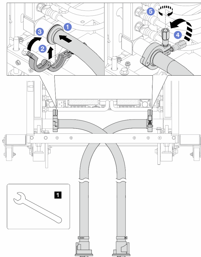
Рис. 173. Установка комплекта шланга
