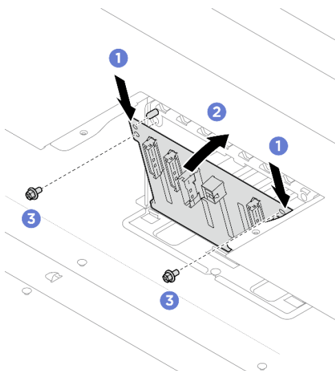
Рис. 25. Установка объединительной панели для 2,5-дюймовых дисков
