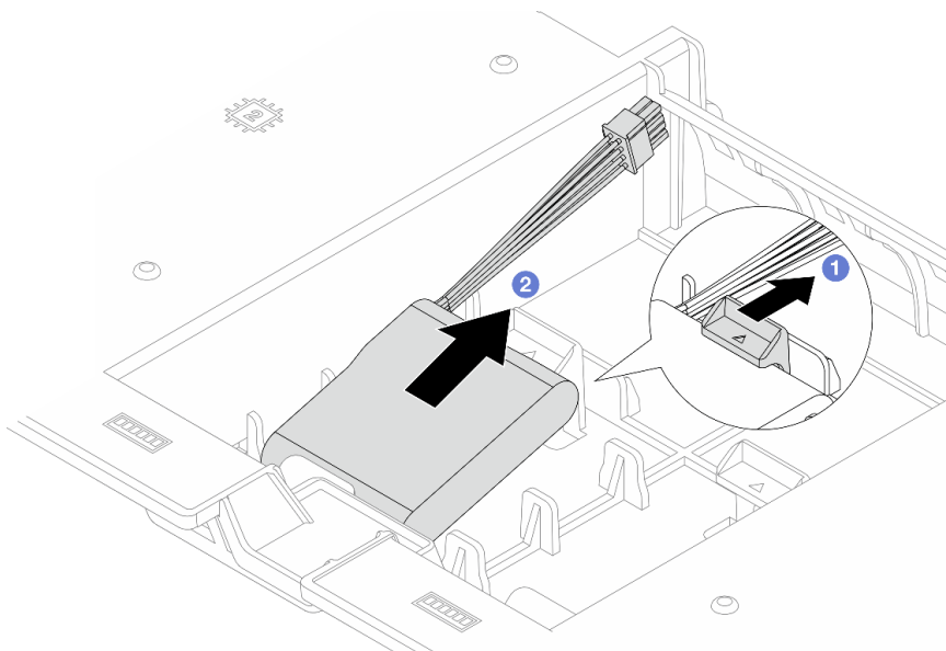
Рис. 206. Снятие модуля питания флэш-памяти RAID с дефлектора
