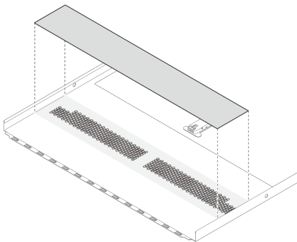
Рис. 244. Майларовая пленка верхнего кожуха
