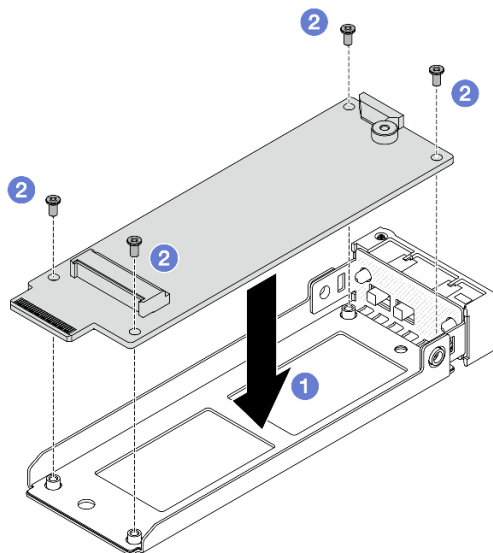
Рис. 115. Установка интерпозера M.2
