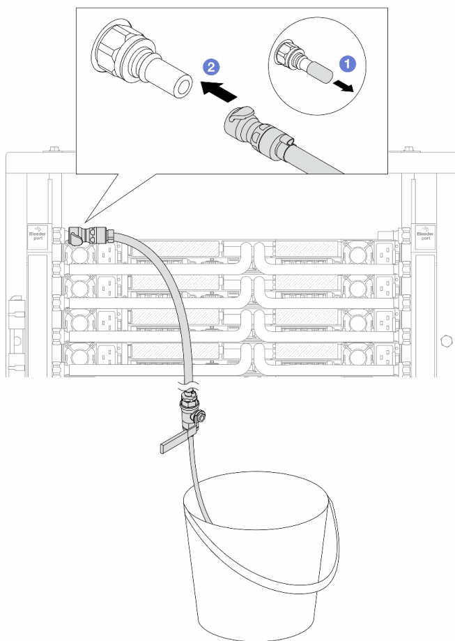
Рис. 157. Установка комплекта отводной трубки на стороне подачи
