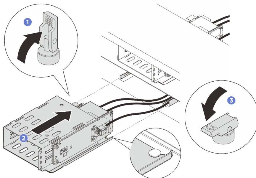
Рис. 51. Установка отсека E3.S 1T
