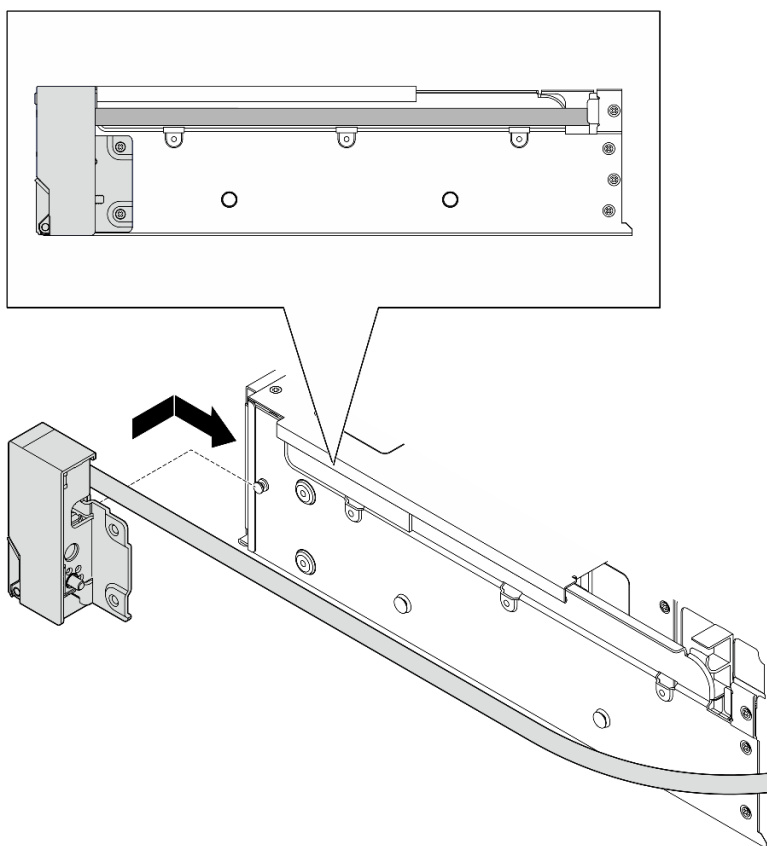
Рис. 202. Установка защелки стойки
