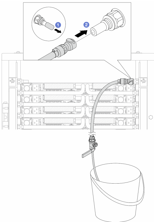
Рис. 160. Установка комплекта отводной трубки на стороне возврата
