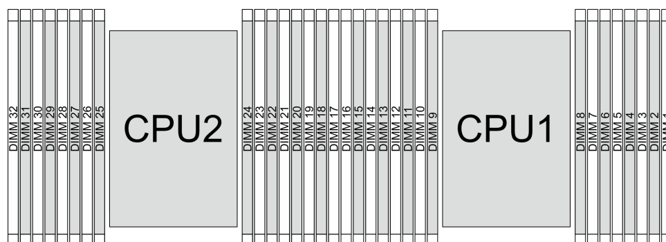
Рис. 1. Гнезда модулей памяти на процессорной плате
