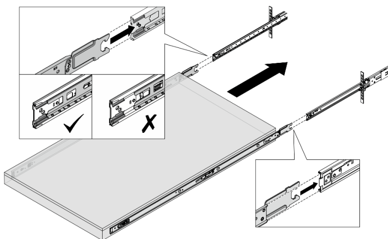
Рис. 14. Взаимоблокировка направляющих
