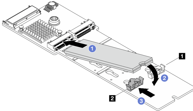
Рис. 81. Установка диска M.2
