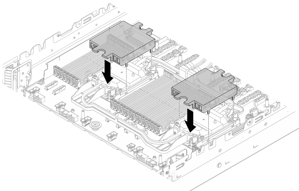
Рис. 99. Установка кожухов плат охлаждения
