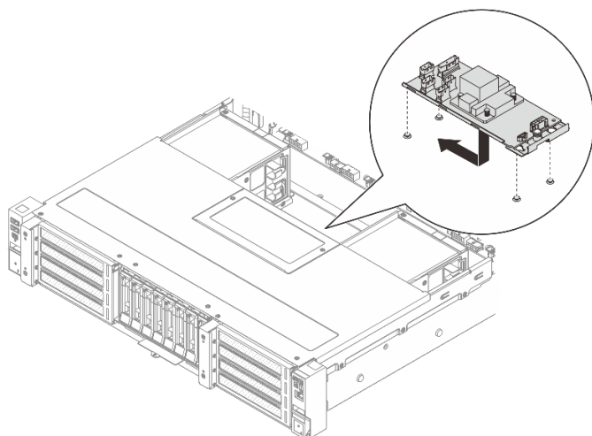
Рис. 77. Установка внутреннего адаптера CFF
