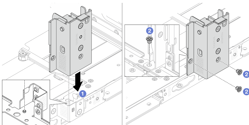
Рис. 222. Установка средней скобы задней стенки
