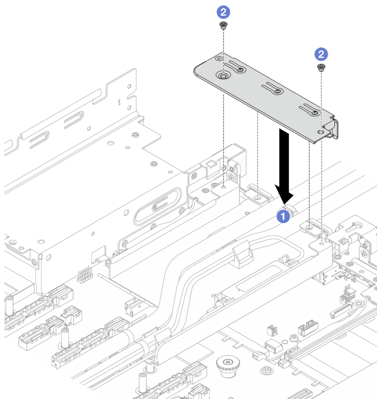
Рис. 102. Установка кронштейна 1FH
