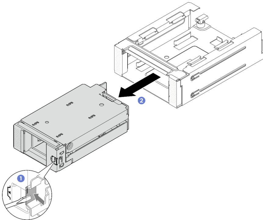
Рис. 119. Снятие переднего отсека для дисков M.2 с корпуса отсека
