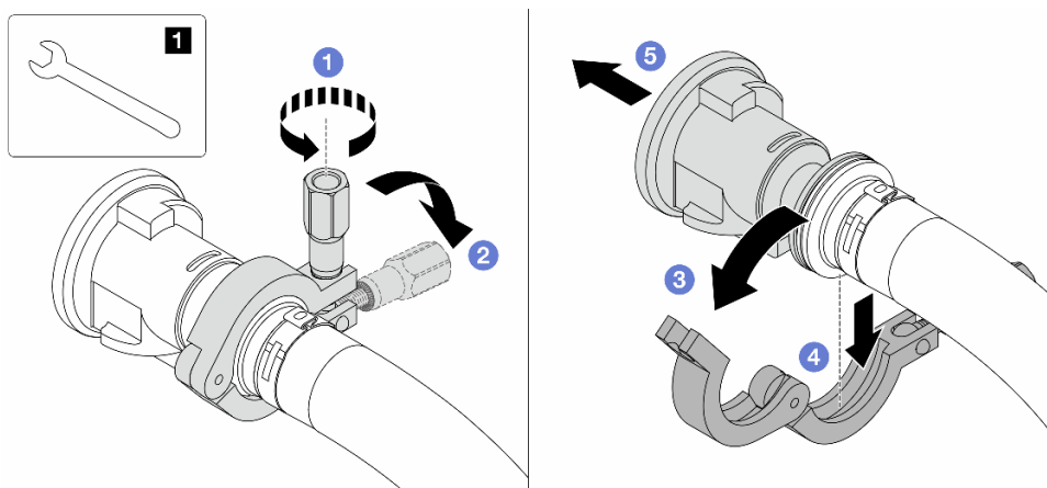
Рис. 150. Отделение шаровых клапанов
