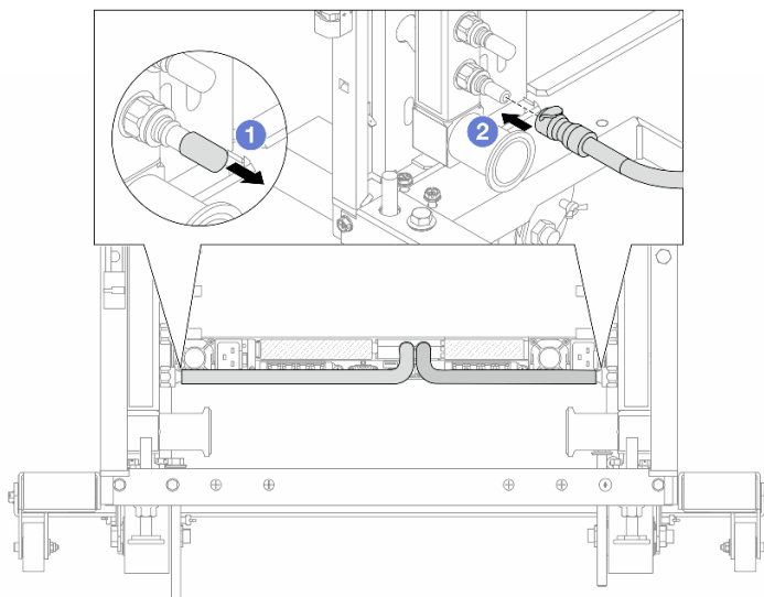
Рис. 172. Установка быстроразъемного соединителя
