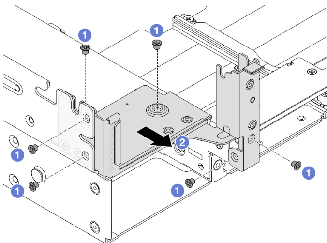
Рис. 218. Снятие левой скобы задней стенки
