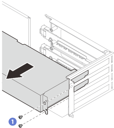
Рис. 54. Снятие адаптера PCIe
