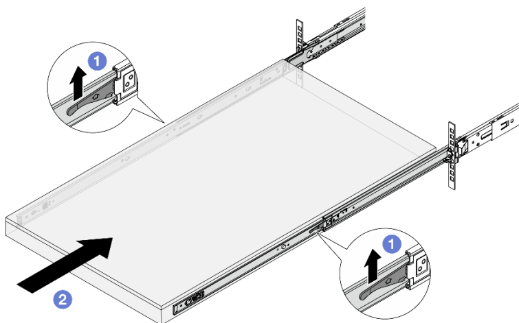
Рис. 15. Блокировка направляющих и установка сервера
