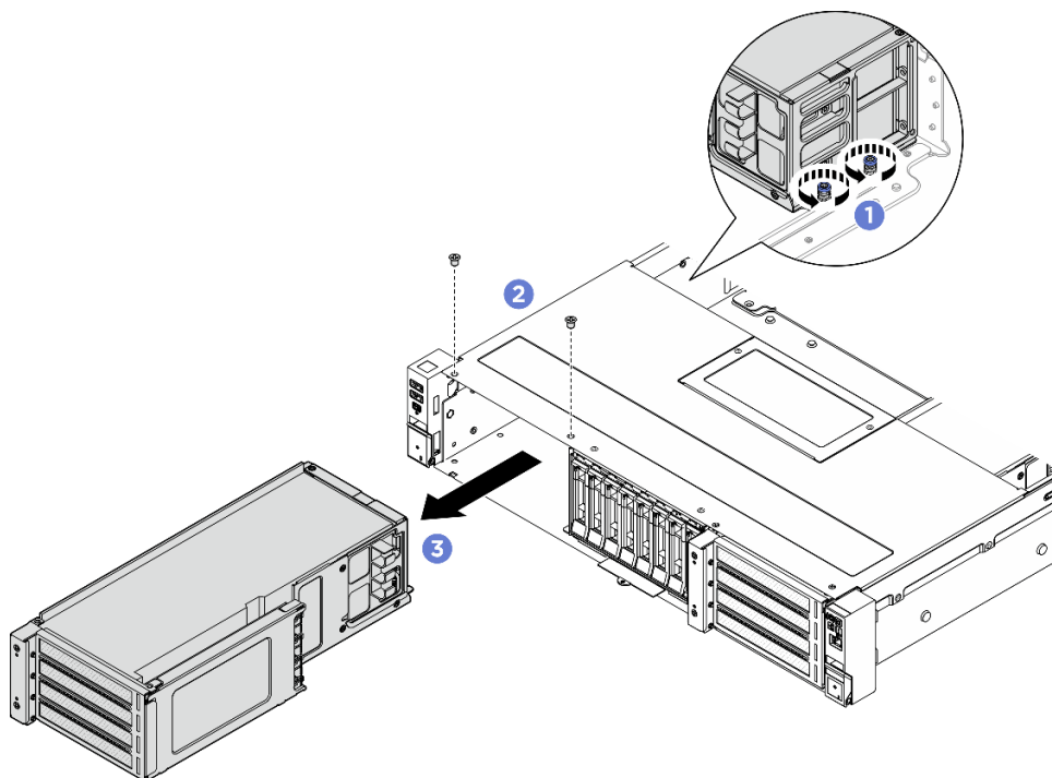
Рис. 52. Снятие переднего блока платы-адаптера Riser
