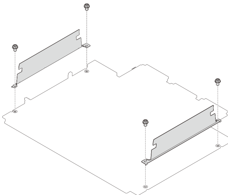
Рис. 34. Установка стенок для кабелей
