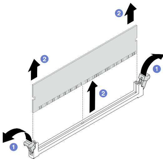
Рис. 182. Снятие модуля памяти
