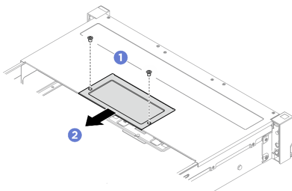
Рис. 21. Снятие защитной панели
