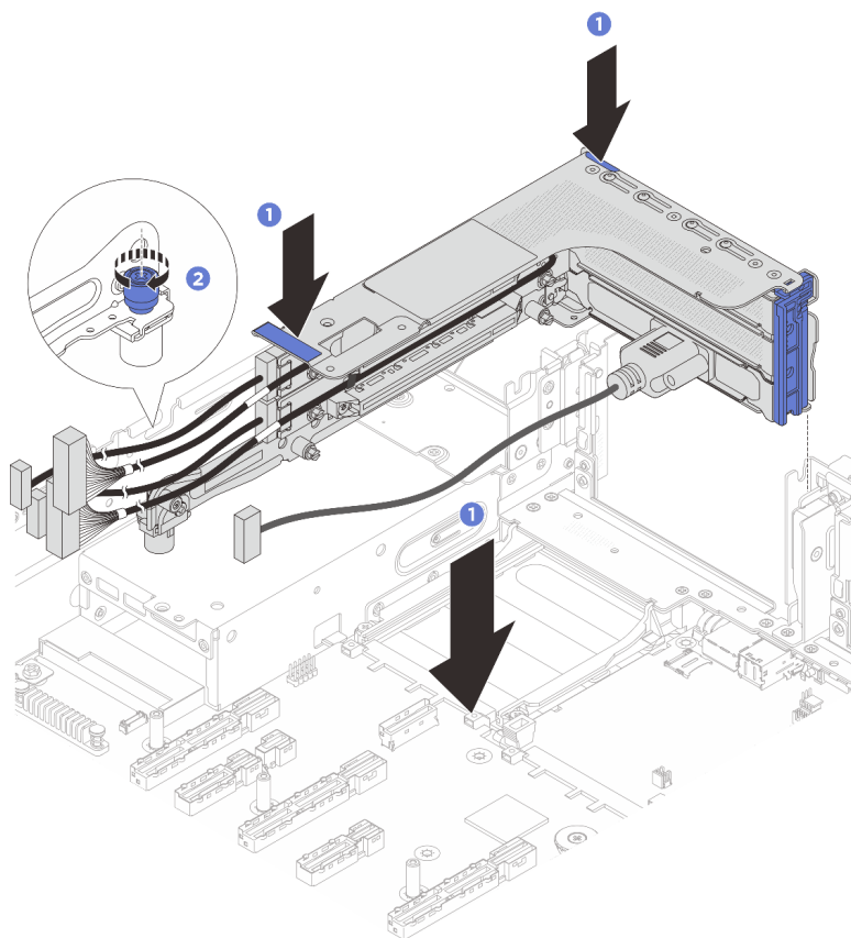
Рис. 229. Установка блока платы-адаптера Riser
