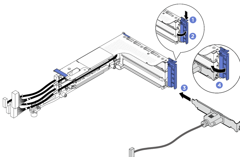
Рис. 228. Установка модуля последовательного порта
