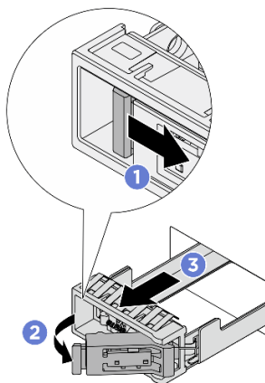
Рис. 107. Снятие лотка для дисков M.2
