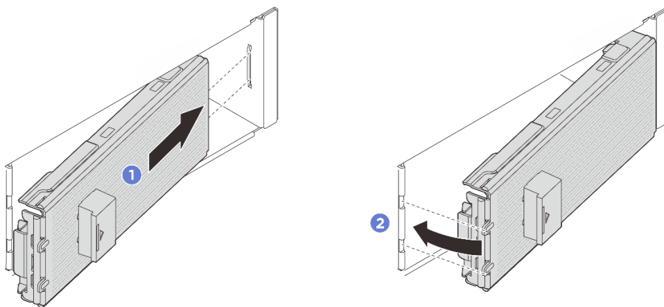
Рис. 44. Установка панели E3.S
