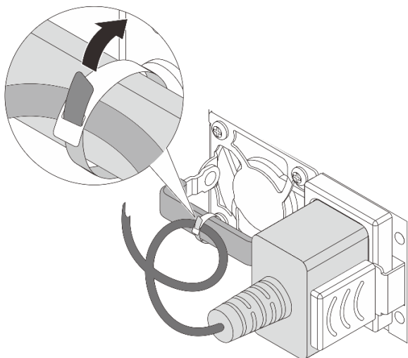
Рис. 74. Прокладка и привязывание шнура питания
