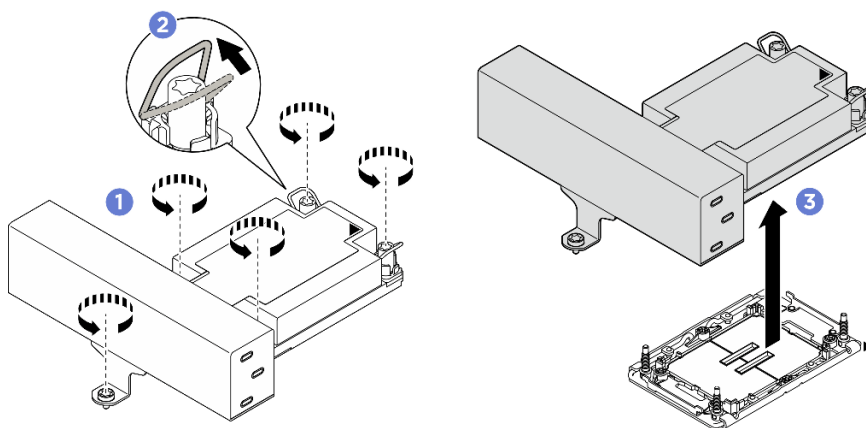
Рис. 188. Снятие T-образного модуля PNM 1U повышенной мощности
