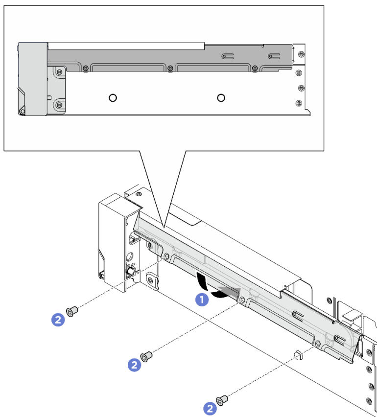
Рис. 204. Установка фиксатора кабелей
