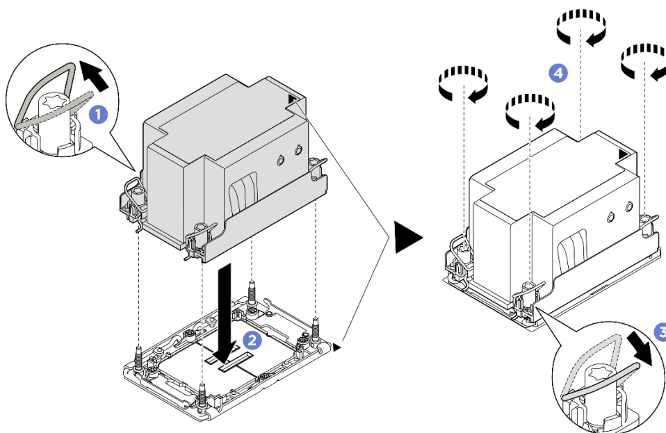
Рис. 197. Установка стандартного PNM 2U
