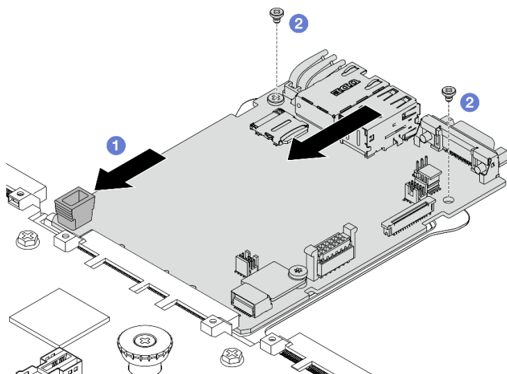
Рис. 237. Установка системной платы ввода-вывода на процессорную плату
