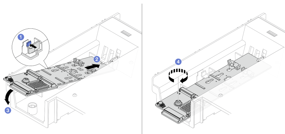
Рис. 84. Установка объединительной панели M.2 на дефлектор
