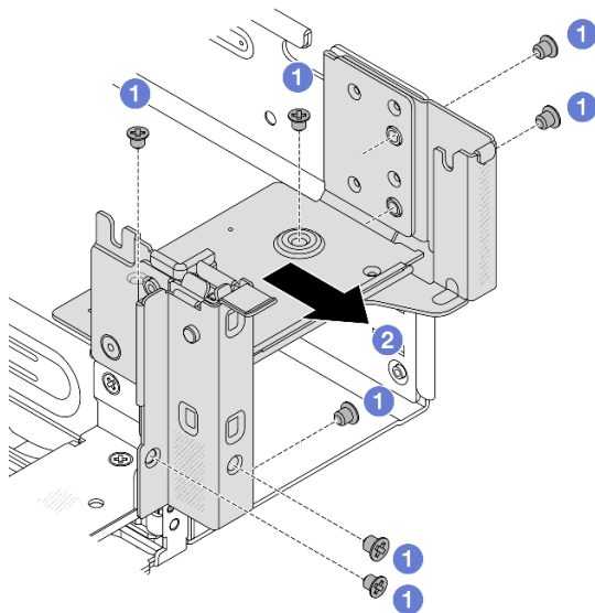
Рис. 220. Снятие правой скобы задней стенки
