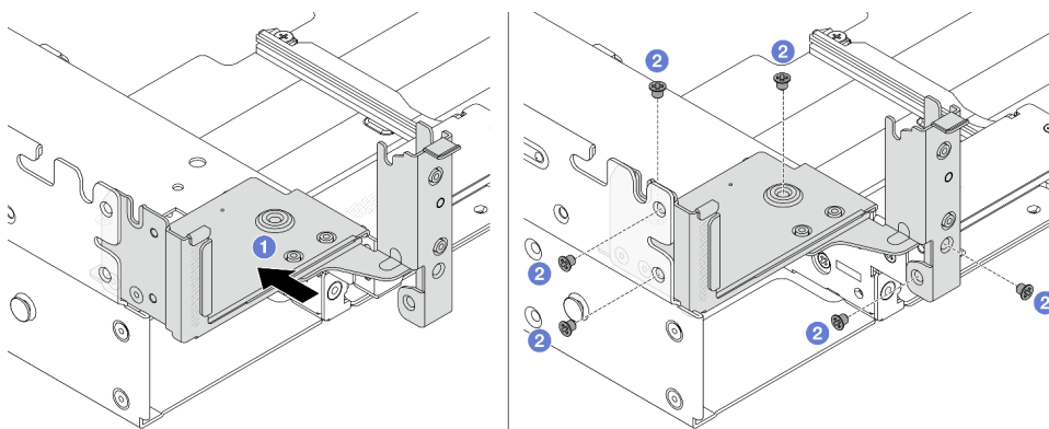
Рис. 221. Установка левой скобы задней стенки
