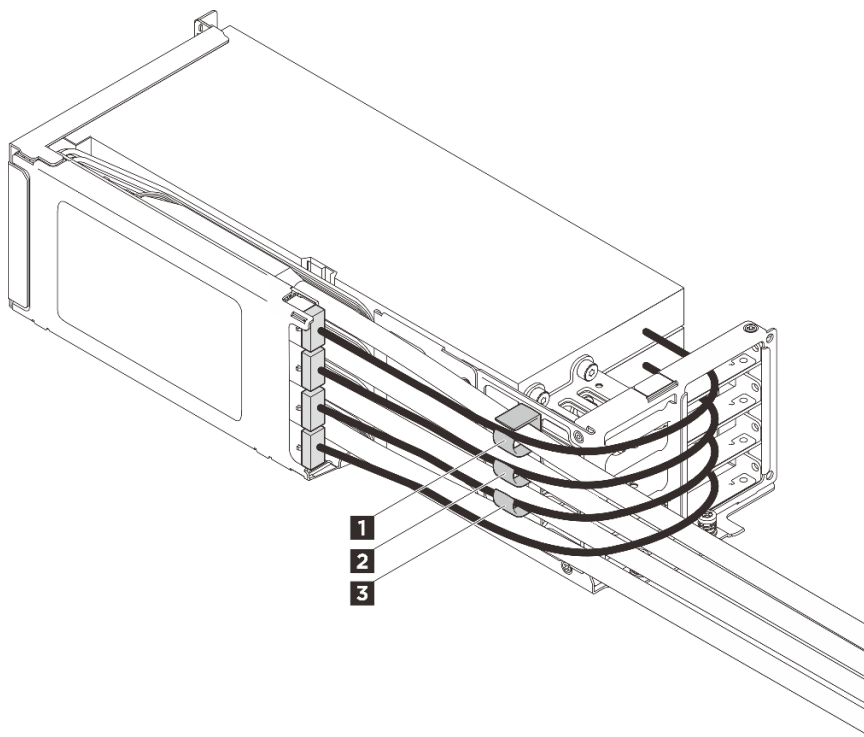
Рис. 64. Кабельные зажимы переднего блока платы-адаптера Riser
