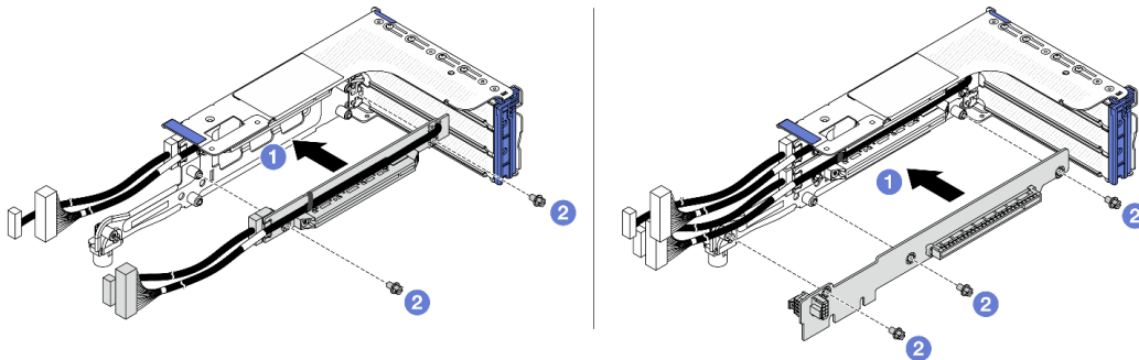
Рис. 215. Установка плат-адаптеров Riser в отсек платы-адаптера 3FH
