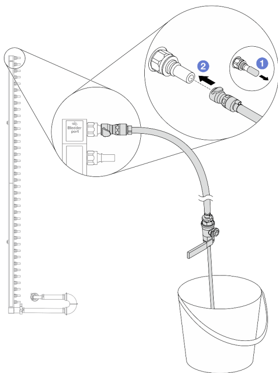
Рис. 144. Установка комплекта отводной трубки на стороне подачи
