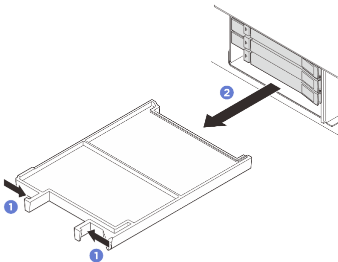
Рис. 40. Снятие заглушки отсека
