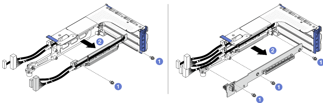
Рис. 214. Снятие плат-адаптеров Riser с отсека платы-адаптера Riser
