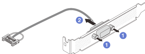
Рис. 226. Разборка модуля последовательного порта
