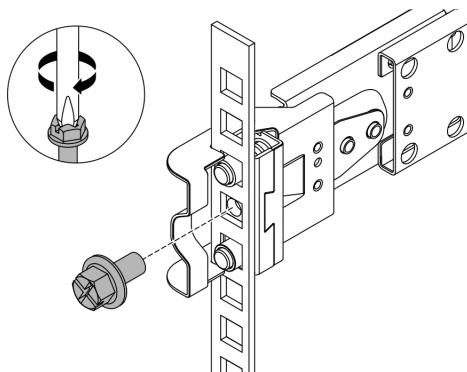
Рис. 17. Фиксация сервера на задней стороне стойки
