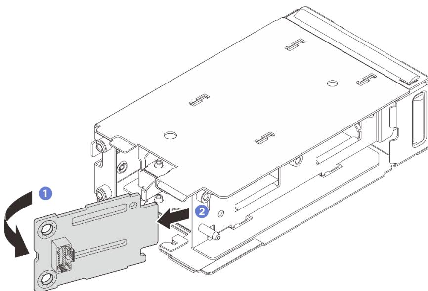
Рис. 122. Снятие передней объединительной панели загрузки M.2
