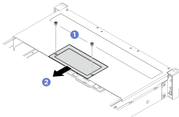
Рис. 45. Снятие защитной пластины
