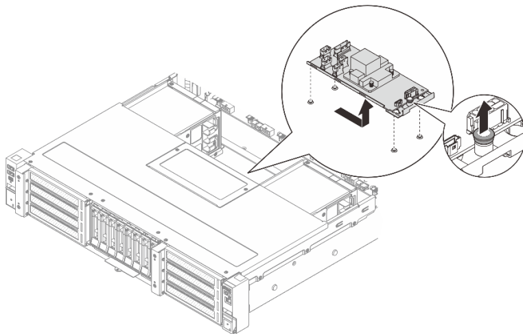
Рис. 76. Снятие внутреннего адаптера CFF
