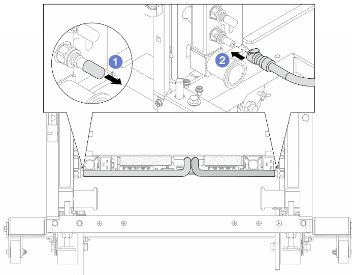
Рис. 156. Установка быстроразъемного соединителя
