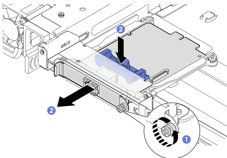
Рис. 132. Снятие адаптера NIC для управления
