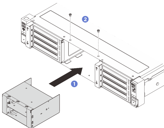
Рис. 49. Установка отсека E3.S
