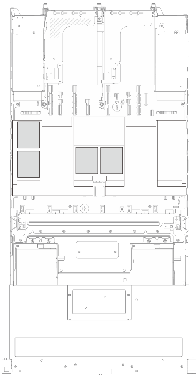
Рис. 205. Расположение модулей питания флэш-памяти RAID на дефлекторе
