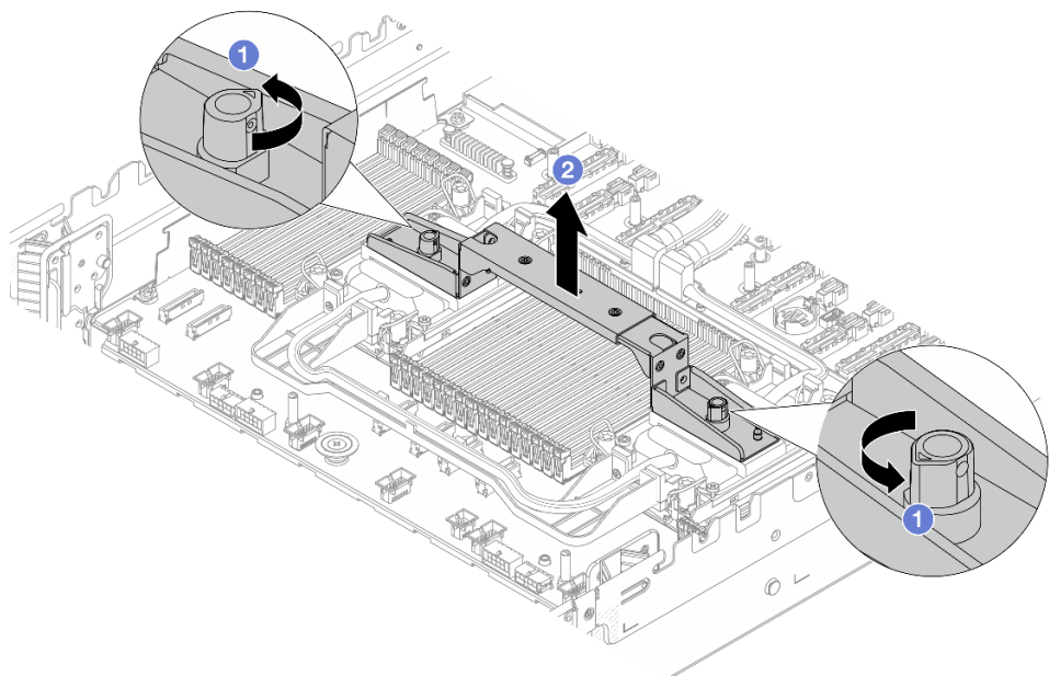
Рис. 98. Снятие ручки модуля
