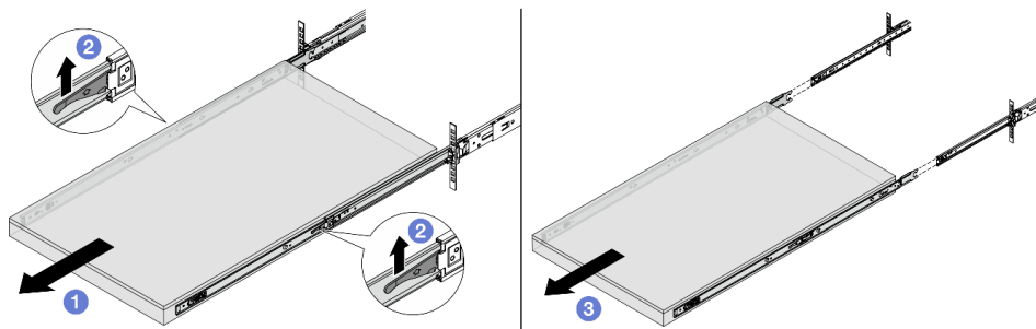
Рис. 9. Извлечение сервера
