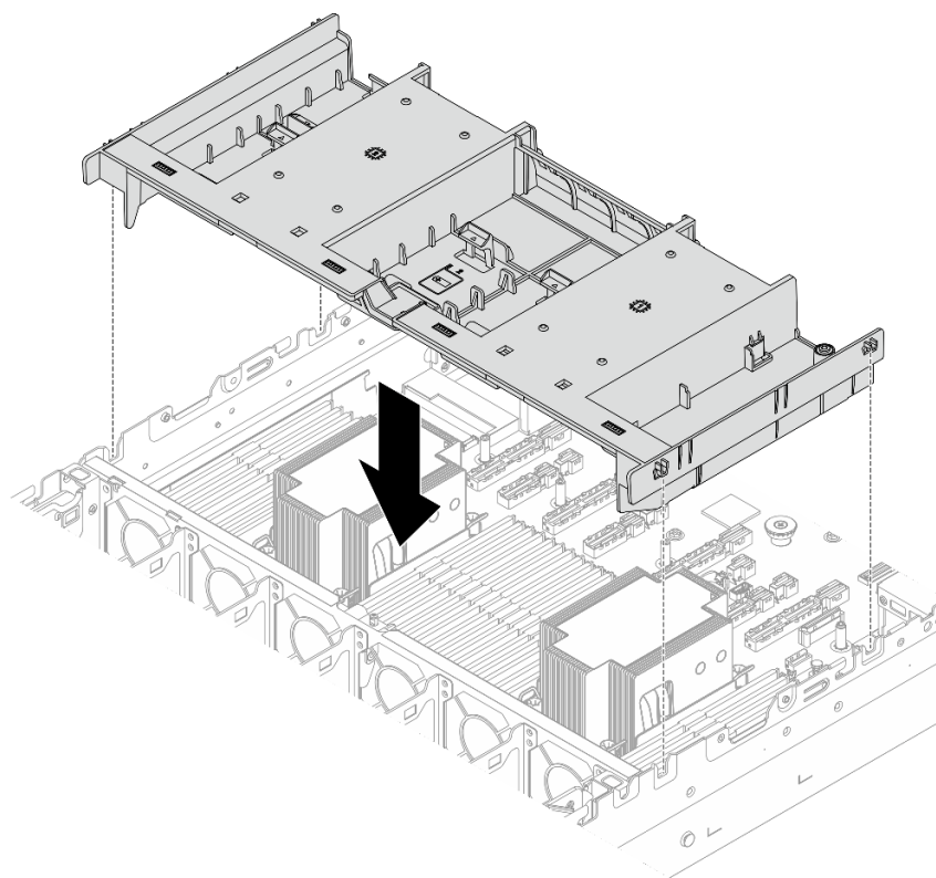
Рис. 31. Установка дефлектора
