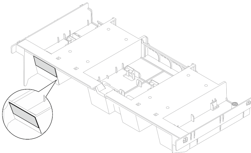
Рис. 30. Майларовый дефлектор
