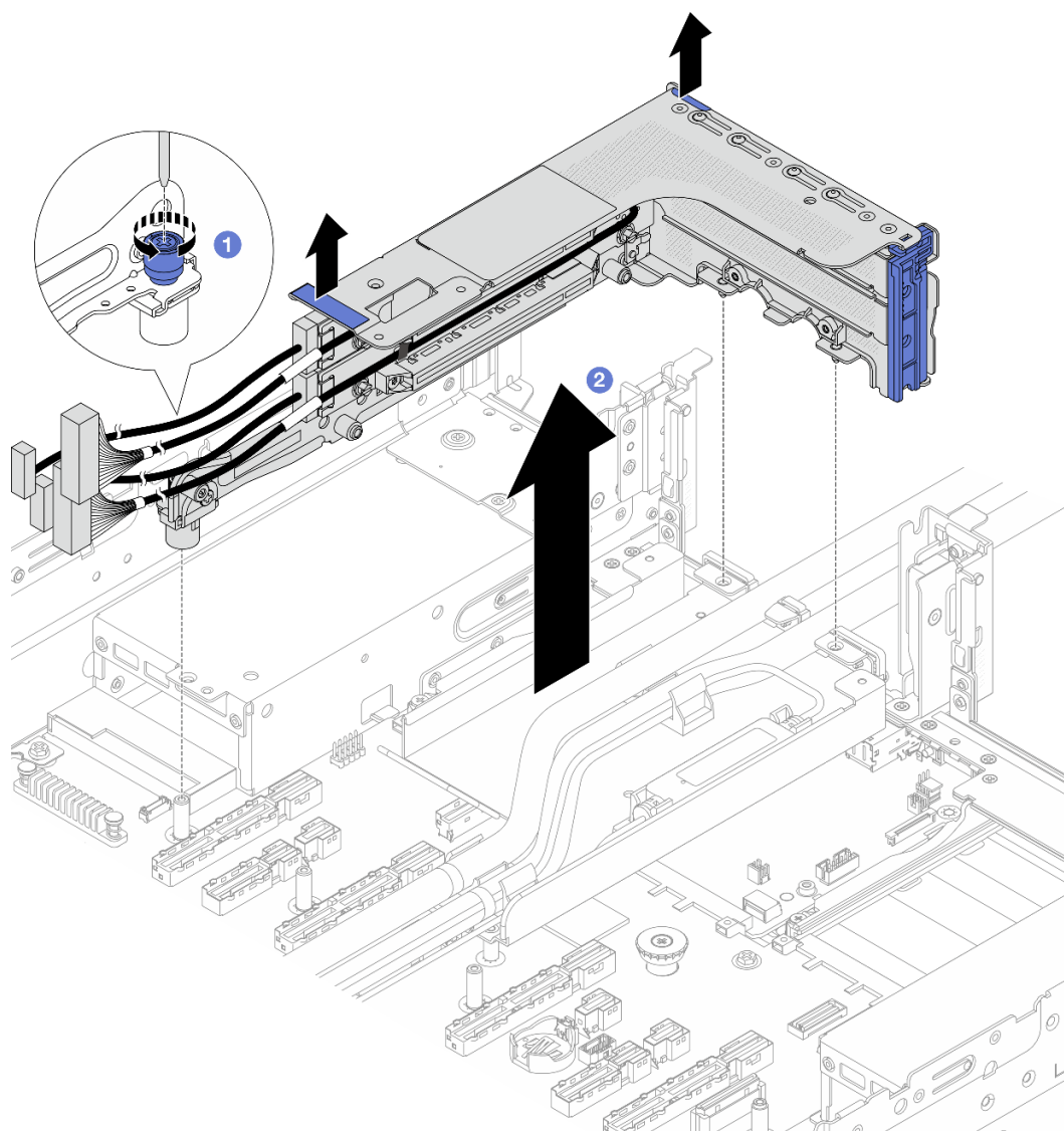
Рис. 90. Снятие отсека платы-адаптера Riser 3FH
