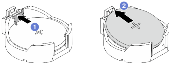
Рис. 35. Снятие батарейки CMOS
