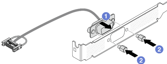
Рис. 227. Сборка модуля последовательного порта
