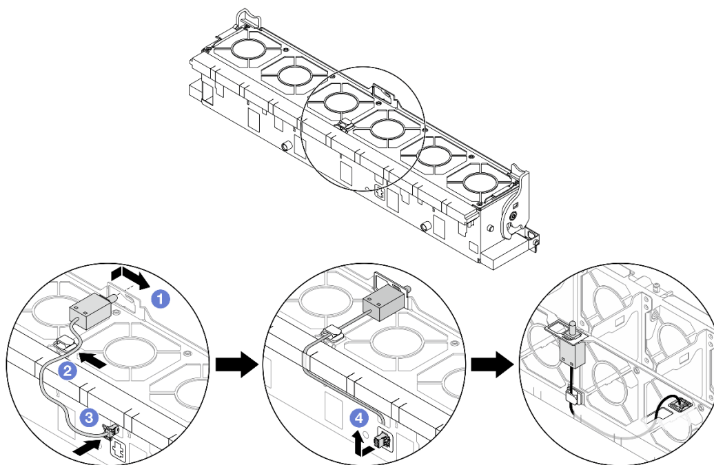
Рис. 88. Установка датчика вмешательства
