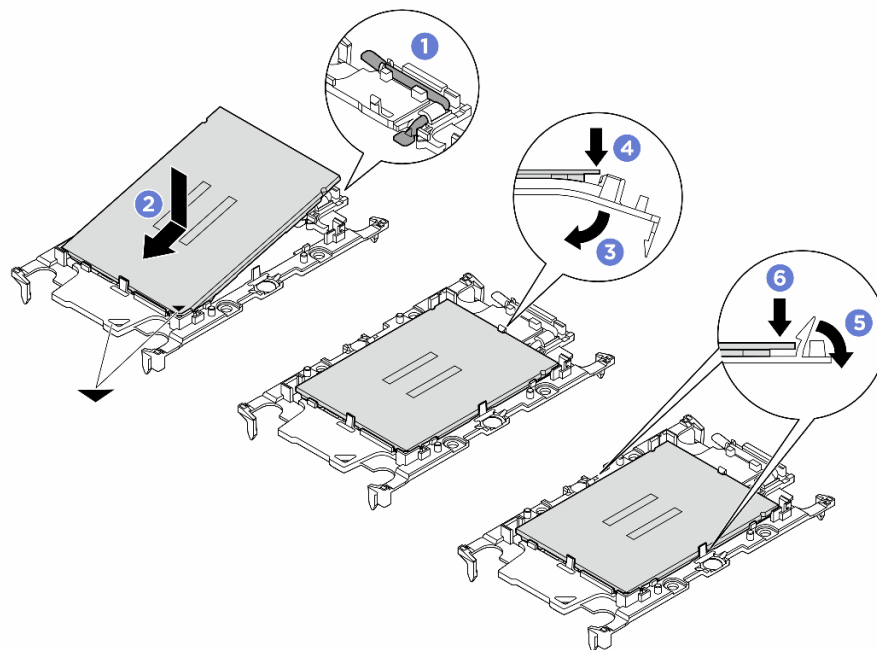
Рис. 193. Установка держателя процессора
