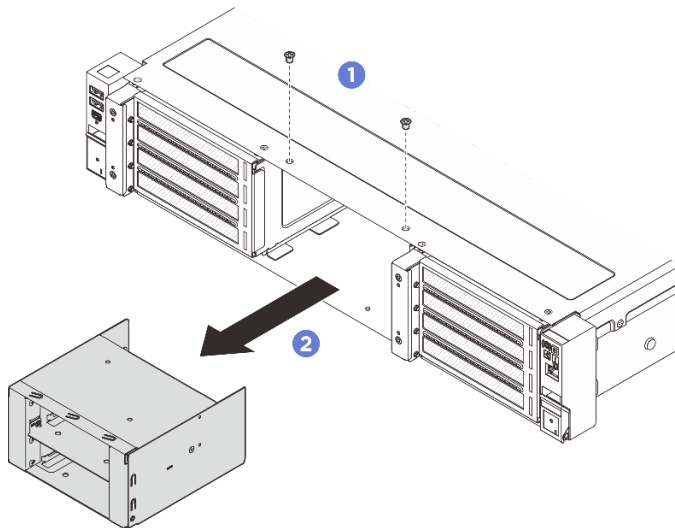
Рис. 48. Снятие отсека для диска E3.S
