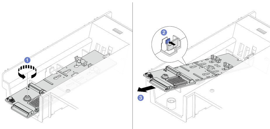
Рис. 83. Снятие объединительной панели M.2 с дефлектора
