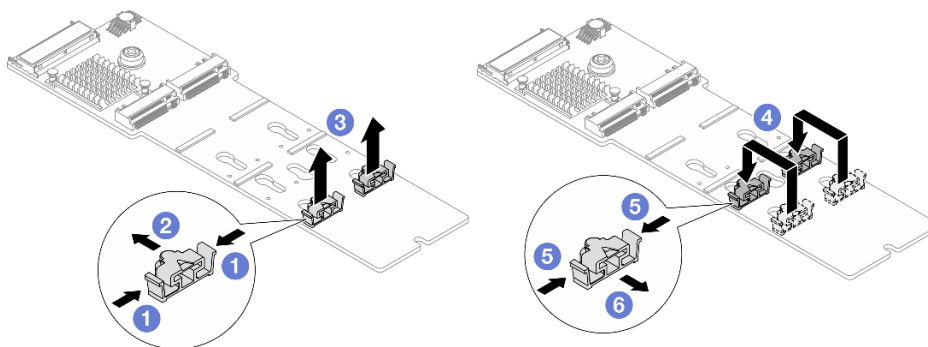
Рис. 79. Регулировка фиксатора M.2
