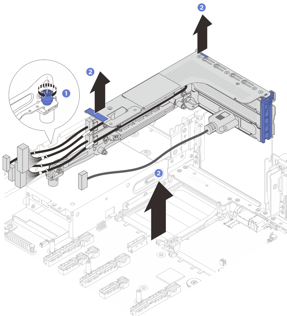
Рис. 224. Снятие блока платы-адаптера Riser
