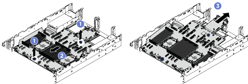
Рис. 231. Снятие блока материнской платы
