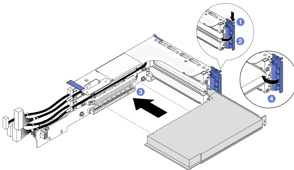
Рис. 216. Установка адаптера PCIe в отсек платы-адаптера Riser 3FH
