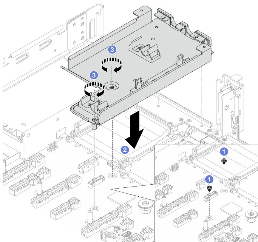
Рис. 94. Установка держателя шланга
