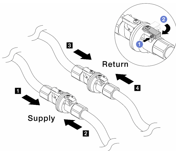
Рис. 181. Открытие шаровых клапанов
