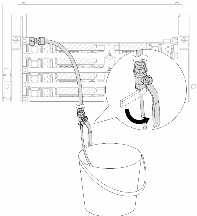
Рис. 180. Открытие клапана отводной трубки на стороне подачи
