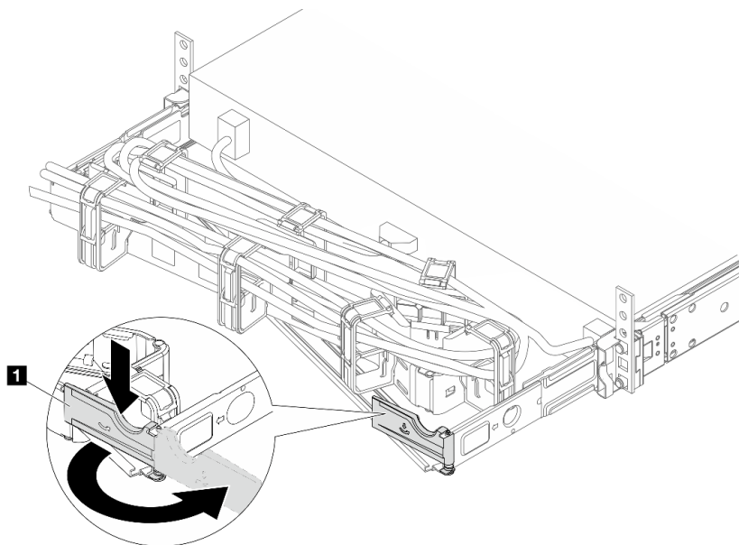
Рис. 67. Регулировка правой стороны
