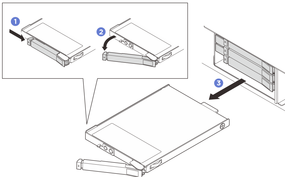
Рис. 38. Снятие оперативно заменяемого диска E3.S
