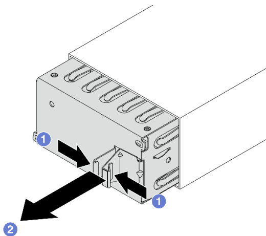
Рис. 72. Снятие заглушки модуля блока питания
