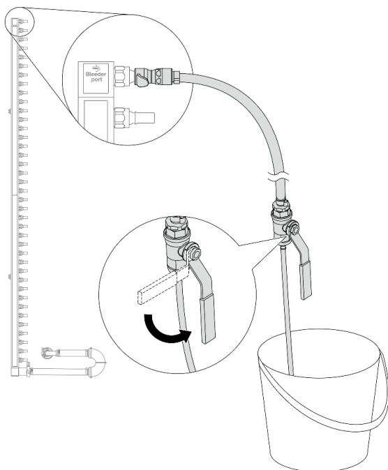
Рис. 145. Открытие клапана отводной трубки
