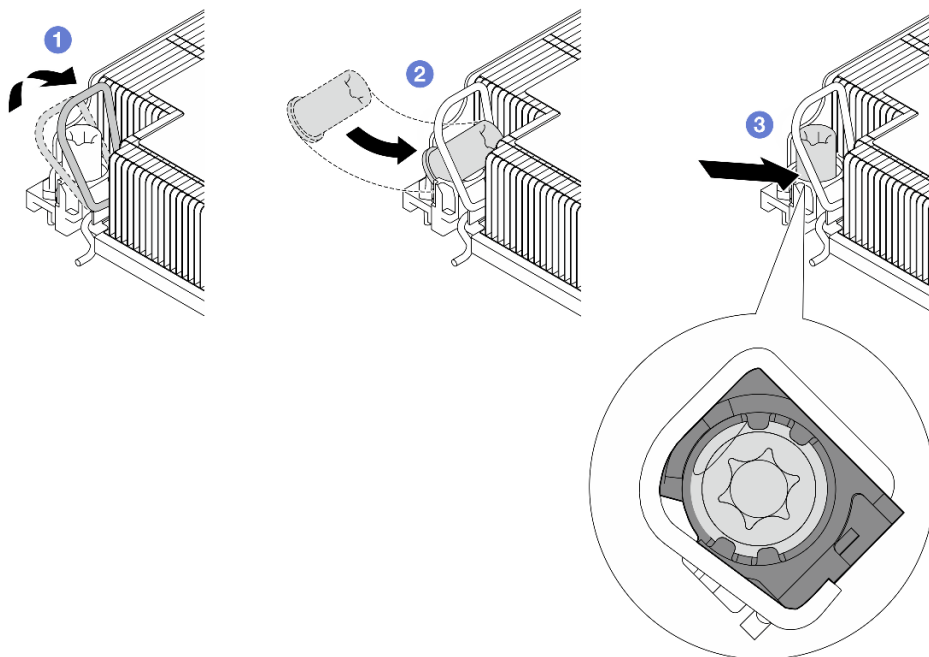
Рис. 66. Установка гайки Torx T30 в радиатор
