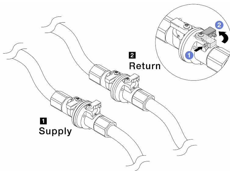
Рис. 163. Закрытие шаровых клапанов
