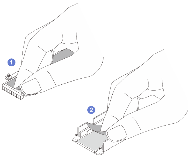
Рис. 113. Снятие пленок
