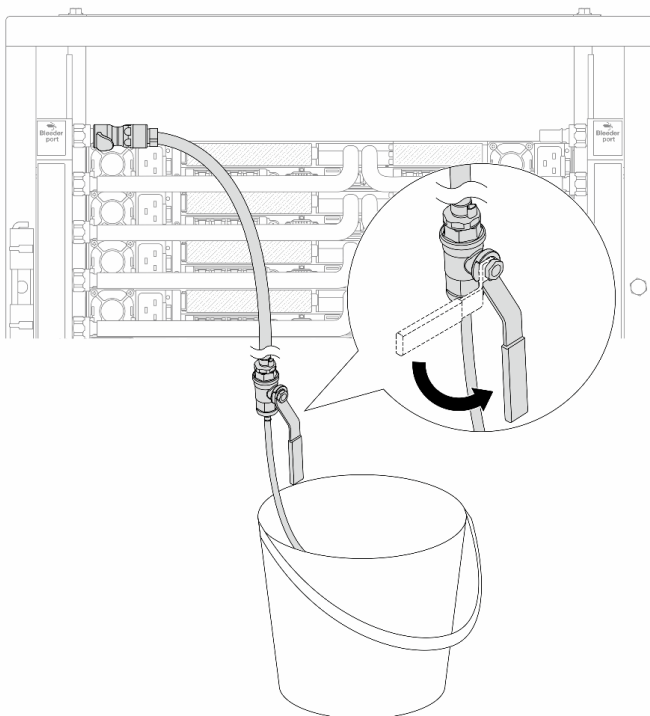
Рис. 162. Открытие клапана отводной трубы на стороне подачи
