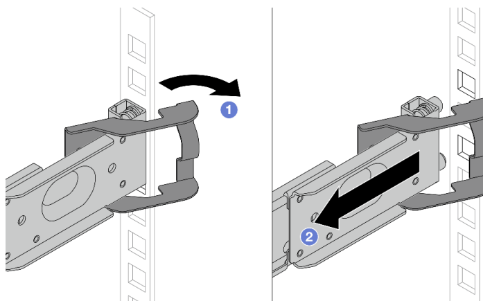
Рис. 4. Снятие направляющей сзади
