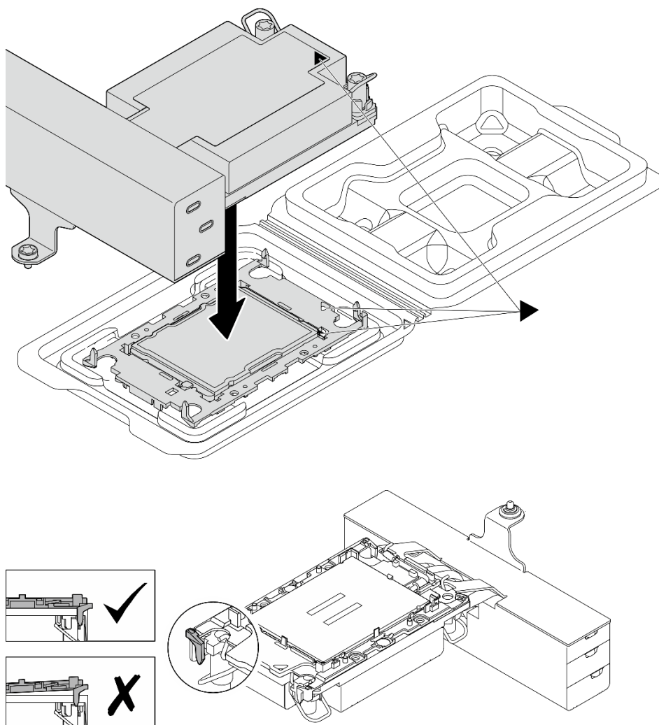
Рис. 195. Сборка модуля процессора с радиатором (PHM), когда процессор находится в транспортировочном лотке
