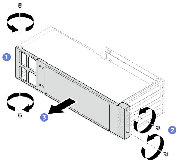
Рис. 53. Снятие боковой опорной скобы
