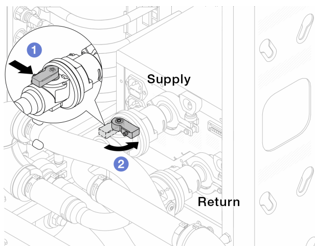
Рис. 140. Закрытие шаровых клапанов
