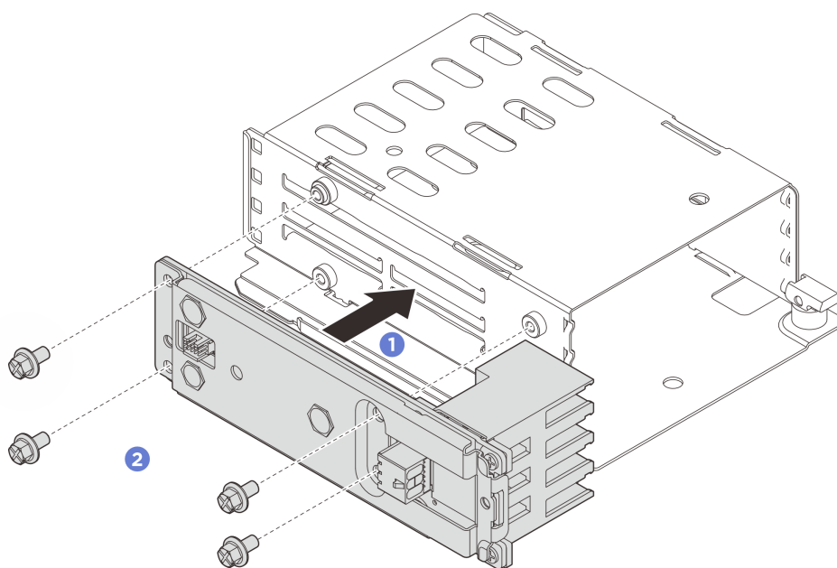
Рис. 50. Установка блока объединительной панели
