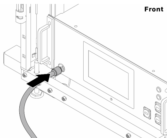
Рис. 154. Передняя сторона блока CDU
