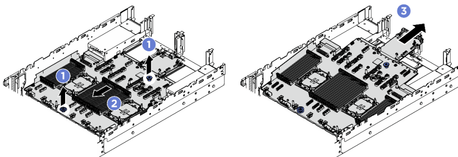
Рис. 235. Снятие блока материнской платы
