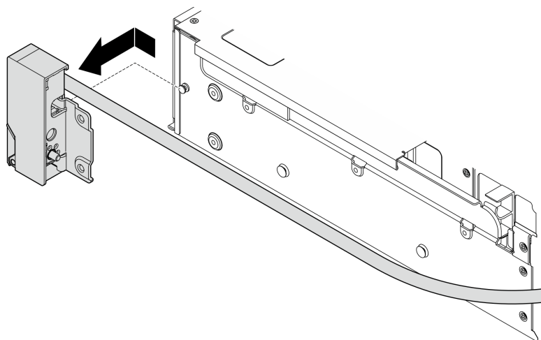
Рис. 201. Снятие защелки стойки
