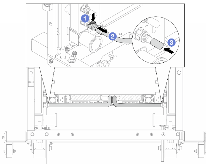
Рис. 141. Отсоединение быстроразъемного соединителя
