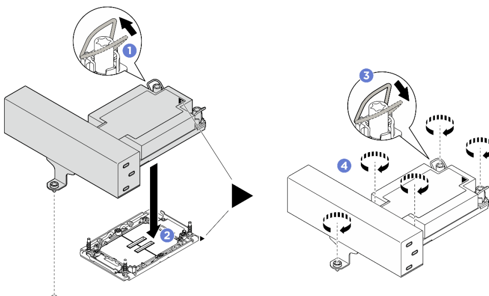
Рис. 198. Установка T-образного PNM 1U повышенной мощности
