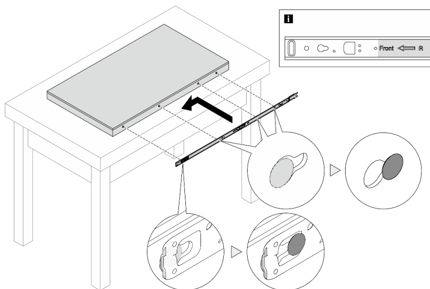
Рис. 12. Установка внутренних направляющих
