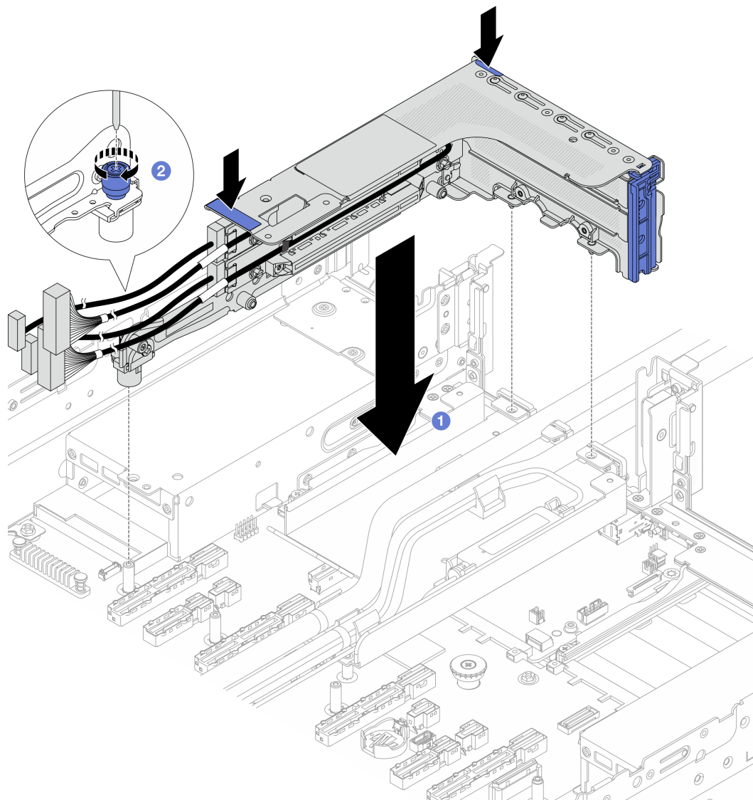
Рис. 103. Установка отсека платы-адаптера Riser 3FH
