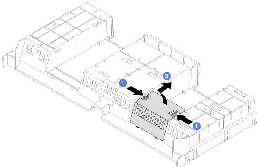
Рис. 28. Снятие заглушки дефлектора
