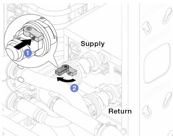
Рис. 158. Открытие шаровых клапанов
