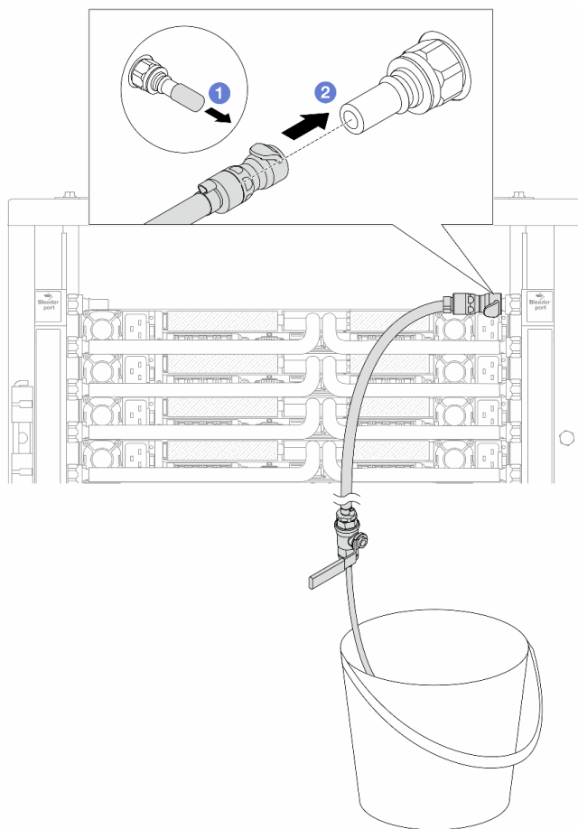
Рис. 177. Установка комплекта отводной трубки на стороне возврата
