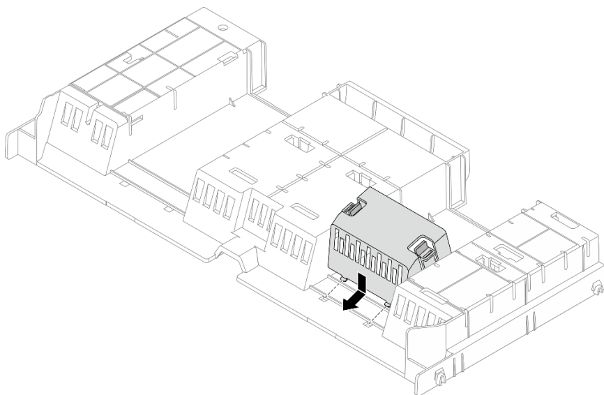
Рис. 29. Установка заглушки дефлектора
