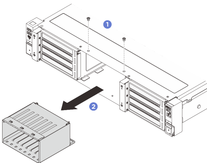
Рис. 23. Снятие отсека для 2,5-дюймовых дисков
