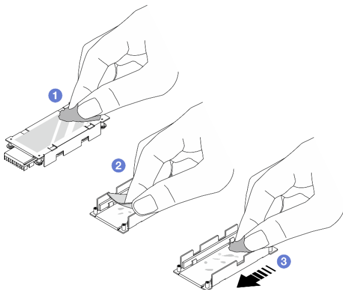
Рис. 112. Очистка радиатора и нижней пластины
