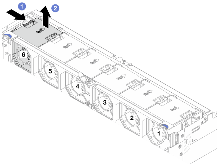
Рис. 239. Снятие вентилятора компьютера
