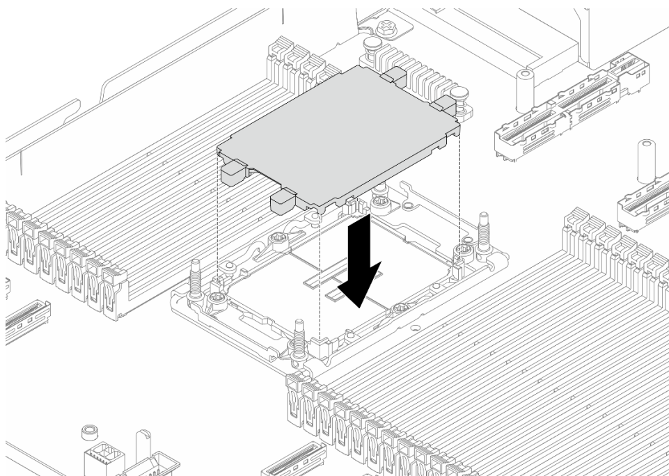
Рис. 96. Установка кожуха гнезда процессора
