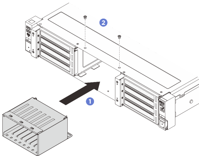
Рис. 24. Установка отсека для 2,5-дюймовых дисков
