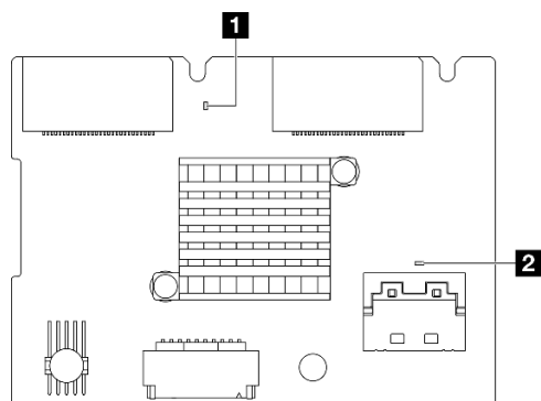
Рис. 257. Светодиодные индикаторы задней объединительной панели M.2
