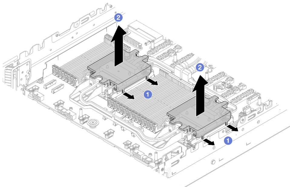
Рис. 264. Снятие кожуха платы охлаждения
