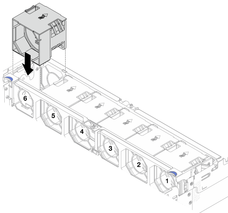
Рис. 240. Установка вентилятора компьютера
