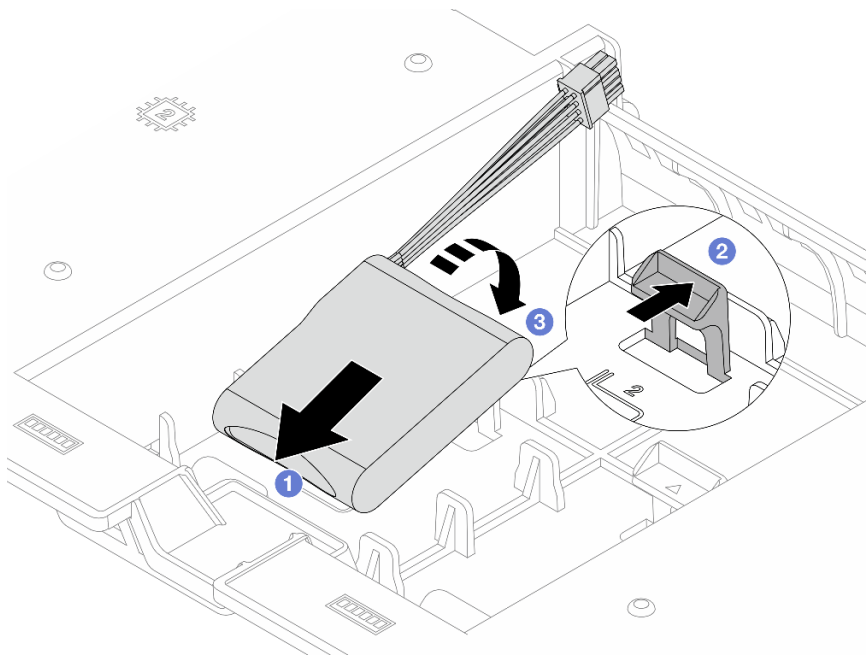
Рис. 207. Установка модуля питания флэш-памяти RAID на дефлектор
