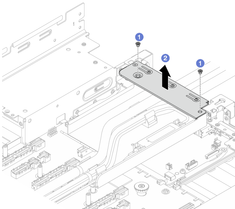
Рис. 89. Снятие скобы 1FH
