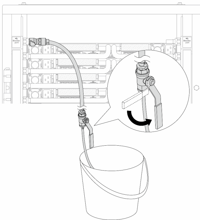
Рис. 176. Открытие клапана отводной трубки на стороне подачи
