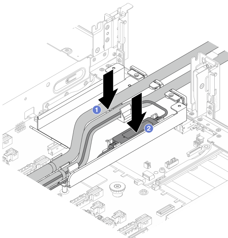
Рис. 100. Размещение шлангов и модуля датчика обнаружения жидкости
