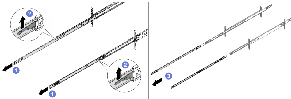
Рис. 11. Выведение направляющих
