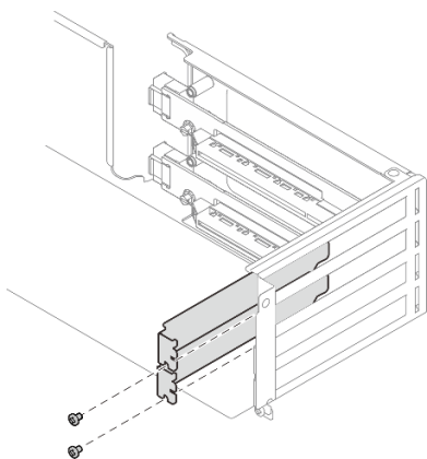
Рис. 56. Заглушка гнезда PCIe
