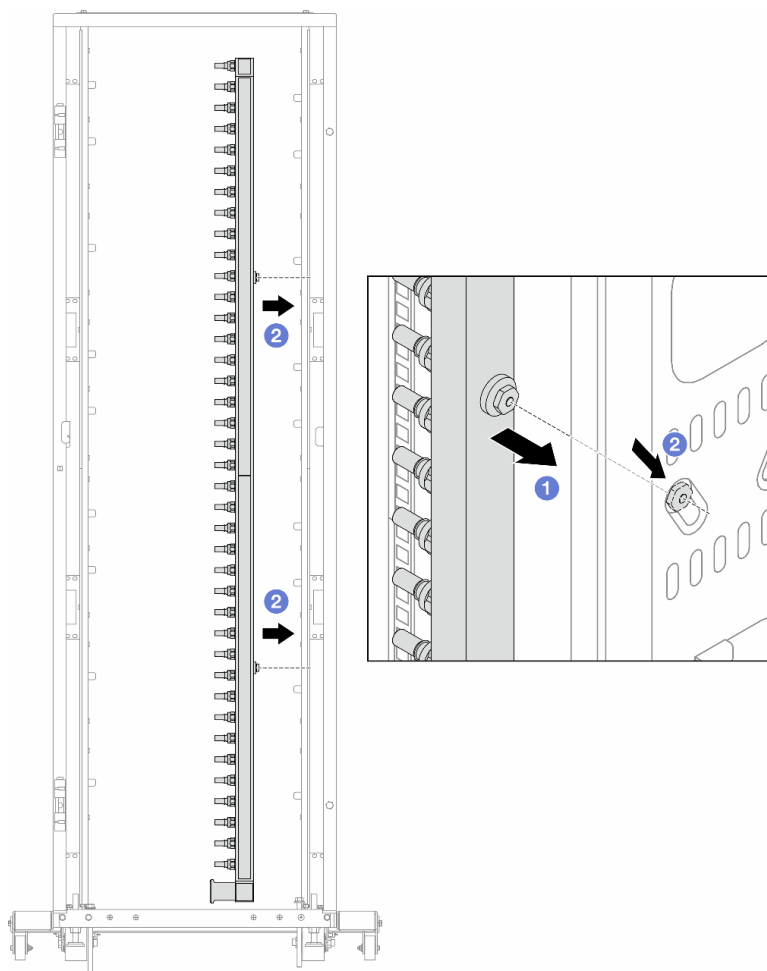
Рис. 171. Установка коллектора
