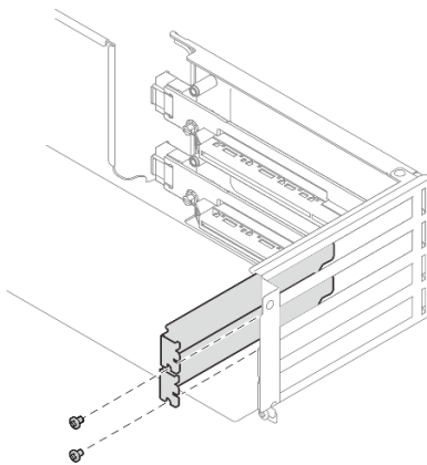
Рис. 55. Заглушка гнезда PCIe
