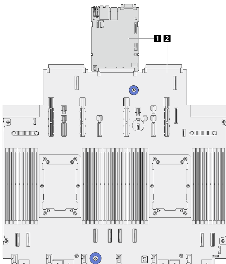
Рис. 230. Компоновка блока материнской платы
