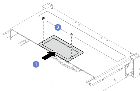
Рис. 26. Установка защитной пластины
