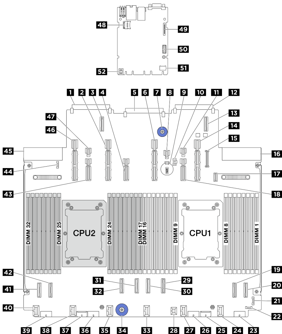
Рис. 250. Разъемы блока материнской платы
