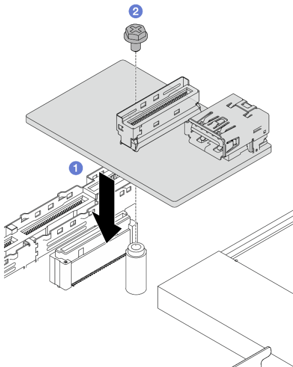
Рис. 247. Установка платы ввода-вывода USB
