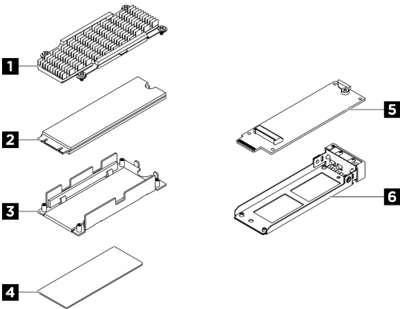
Рис. 104. Компоненты блока оперативно заменяемых дисков M.2
