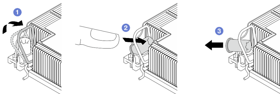
Рис. 65. Снятие гайки Torx T30 с радиатора
