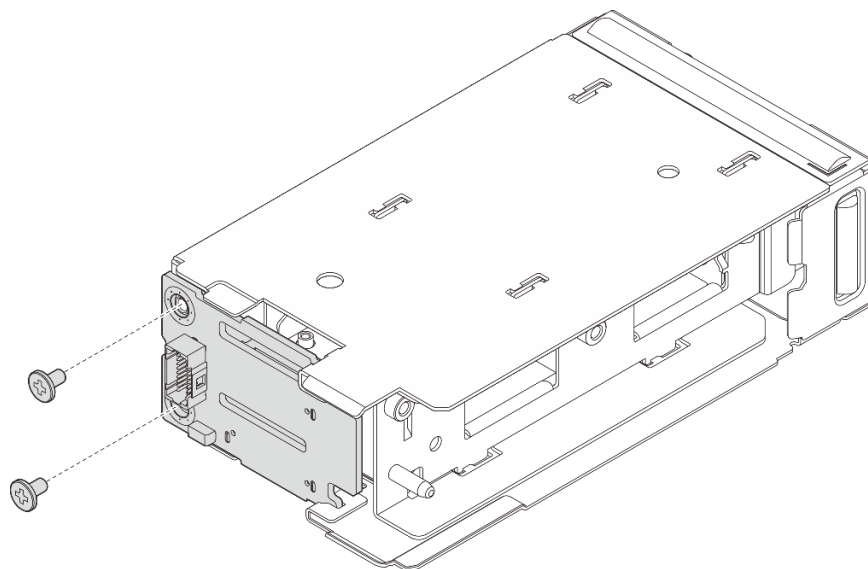
Рис. 121. Снятие передней объединительной панели загрузки M.2
