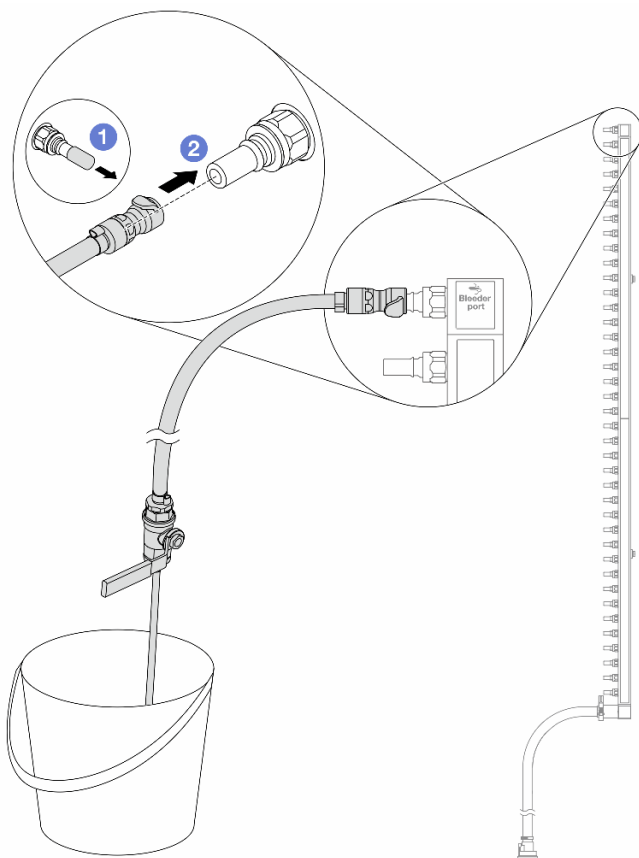
Рис. 168. Установка комплекта отводной трубки на стороне возврата
