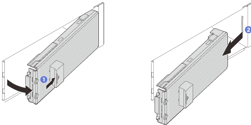
Рис. 37. Снятие панели E3.S
