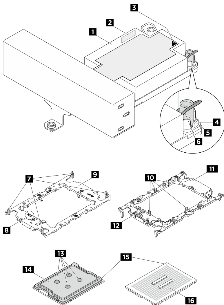
Рис. 186. Компоненты PHM
