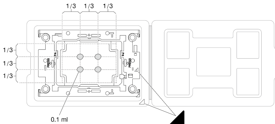
Рис. 194. Нанесение термопасты на процессор в транспортировочном лотке
