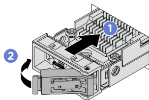
Рис. 108. Установка блока дисков M.2
