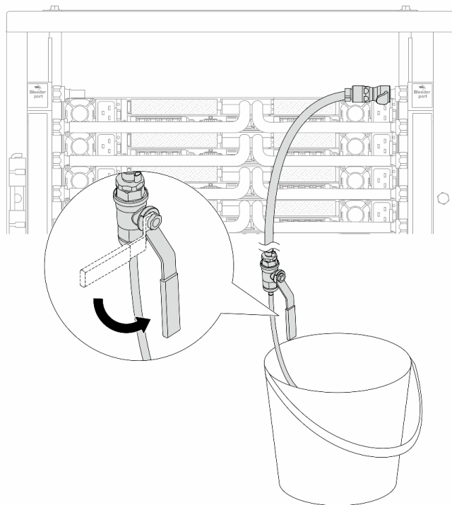
Рис. 179. Открытие клапана отводной трубки на стороне возврата
