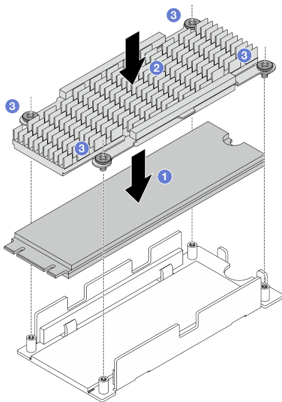
Рис. 114. Установка диска M.2
