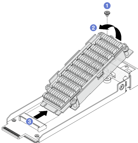
Рис. 109. Снятие диска M.2 с радиатором
