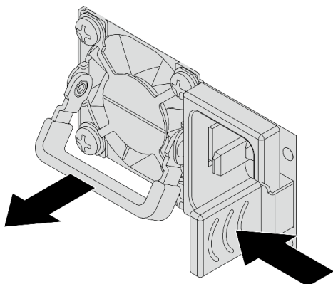
Рис. 69. Снятие оперативно заменяемого модуля блока питания
