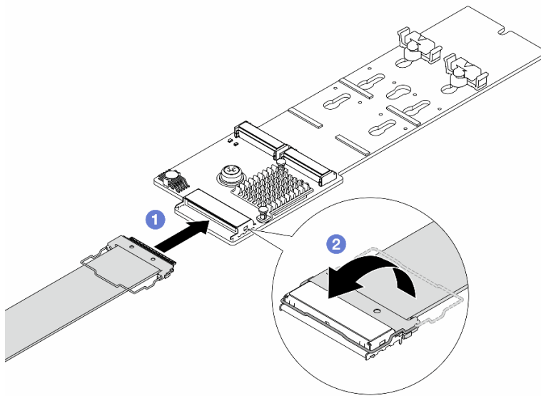
Рис. 85. Подключение кабеля M.2
