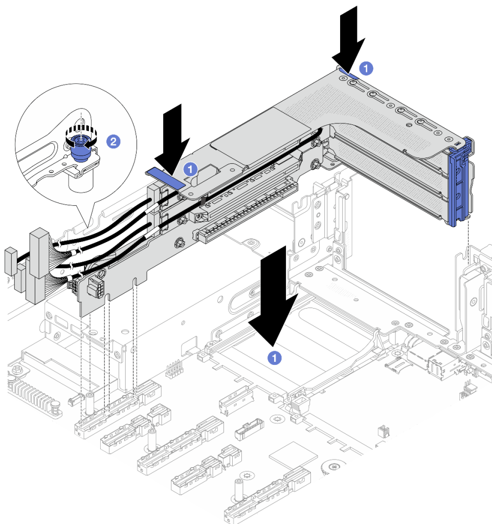
Рис. 217. Установка блока платы-адаптера Riser 3FH
