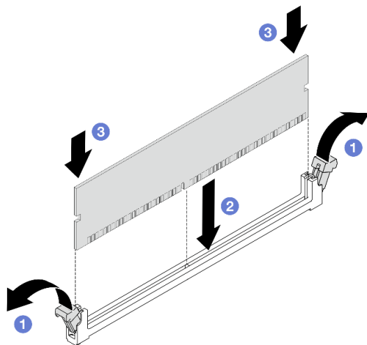
Рис. 183. Установка модуля памяти
