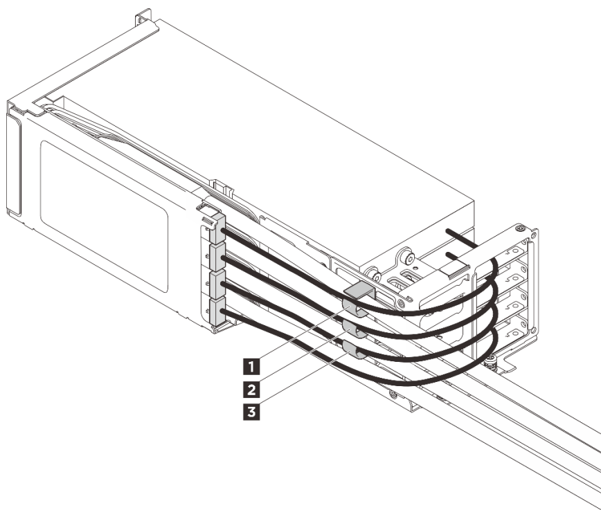
Рис. 61. Кабельные зажимы переднего блока платы-адаптера Riser
