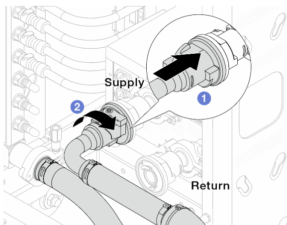
Рис. 153. Подключение шаровых клапанов
