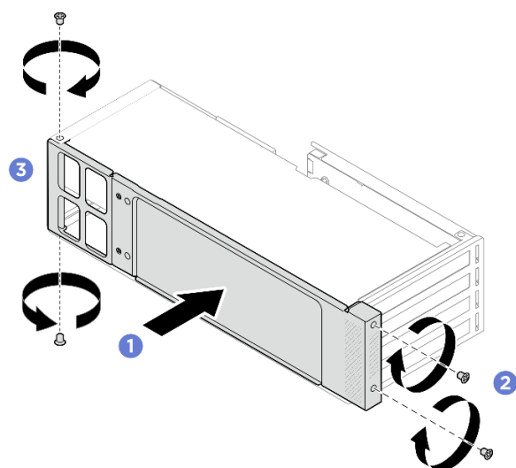
Рис. 59. Установка боковой опорной скобы
