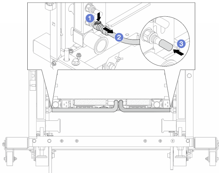
Рис. 164. Отсоединение быстроразъемного соединителя
