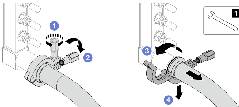
Рис. 148. Отделение коллектора от комплекта соединений
