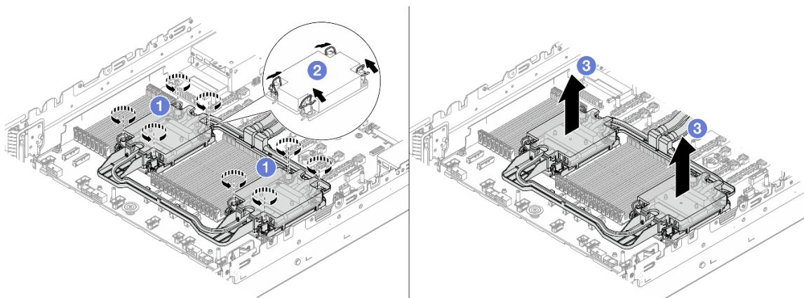
Рис. 92. Снятие Processor Neptune Core Module
