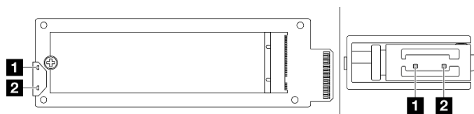
Рис. 256. Светодиодные индикаторы интерпозера М.2
