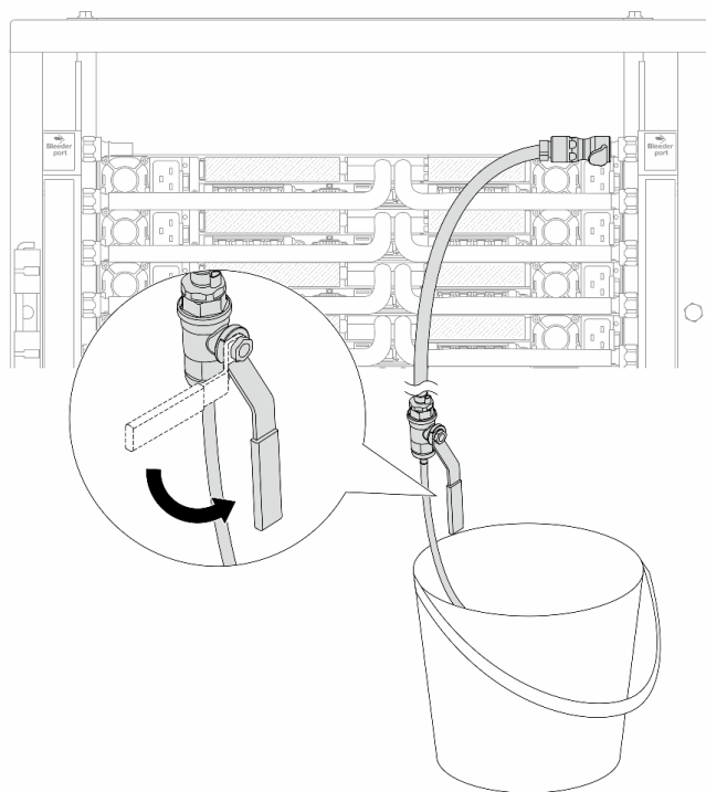
Рис. 161. Открытие клапана отводной трубки на стороне возврата
