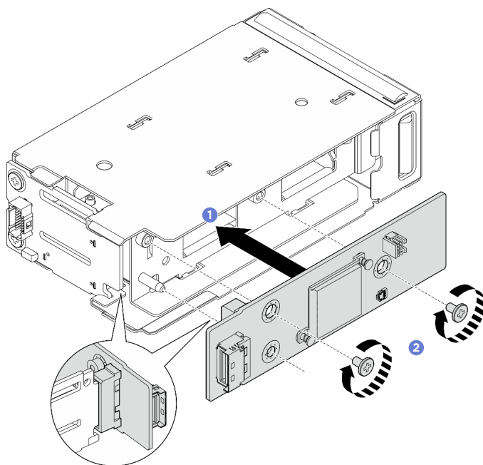
Рис. 126. Установка передней платы контроллера M.2
