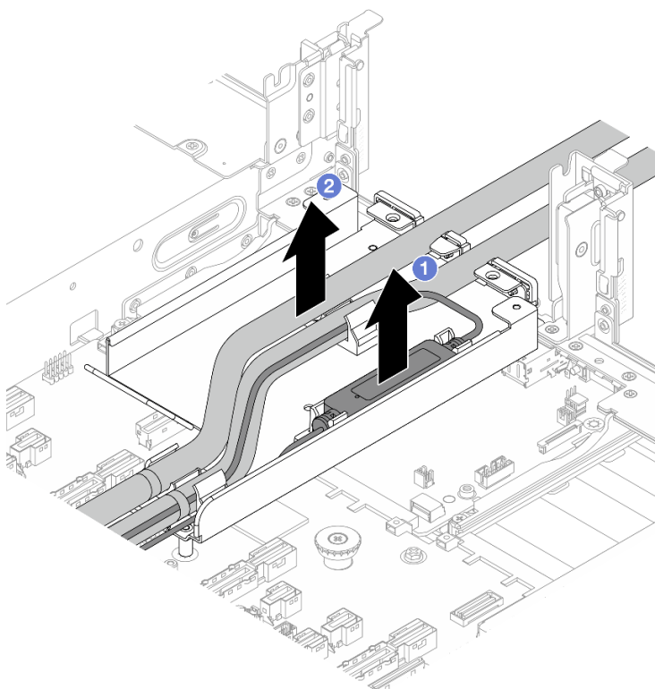
Рис. 91. Отсоединение шлангов и компонента «модуль датчика обнаружения жидкости»
