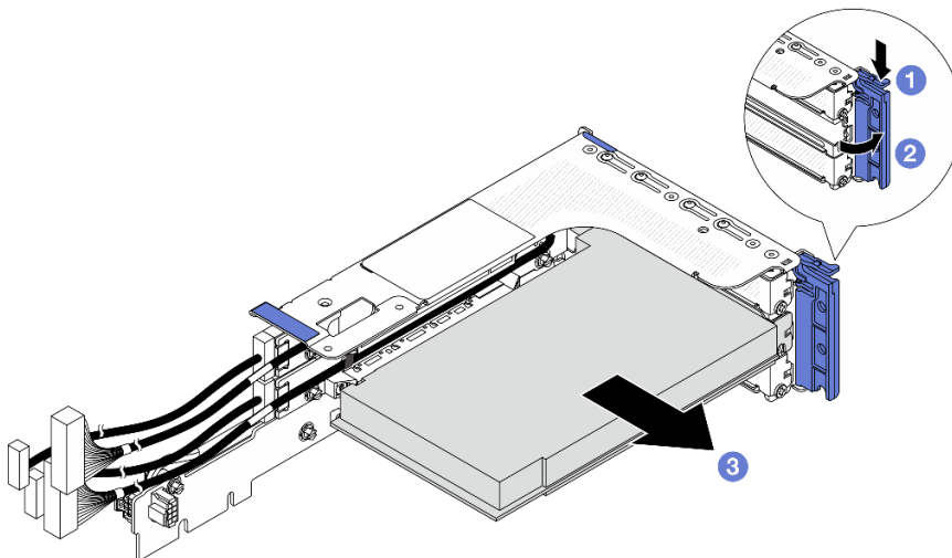
圖例 227. 從 3FH 擴充卡匣卸下 PCIe 配接卡
