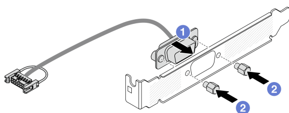
圖例 241. 組裝序列埠模組
