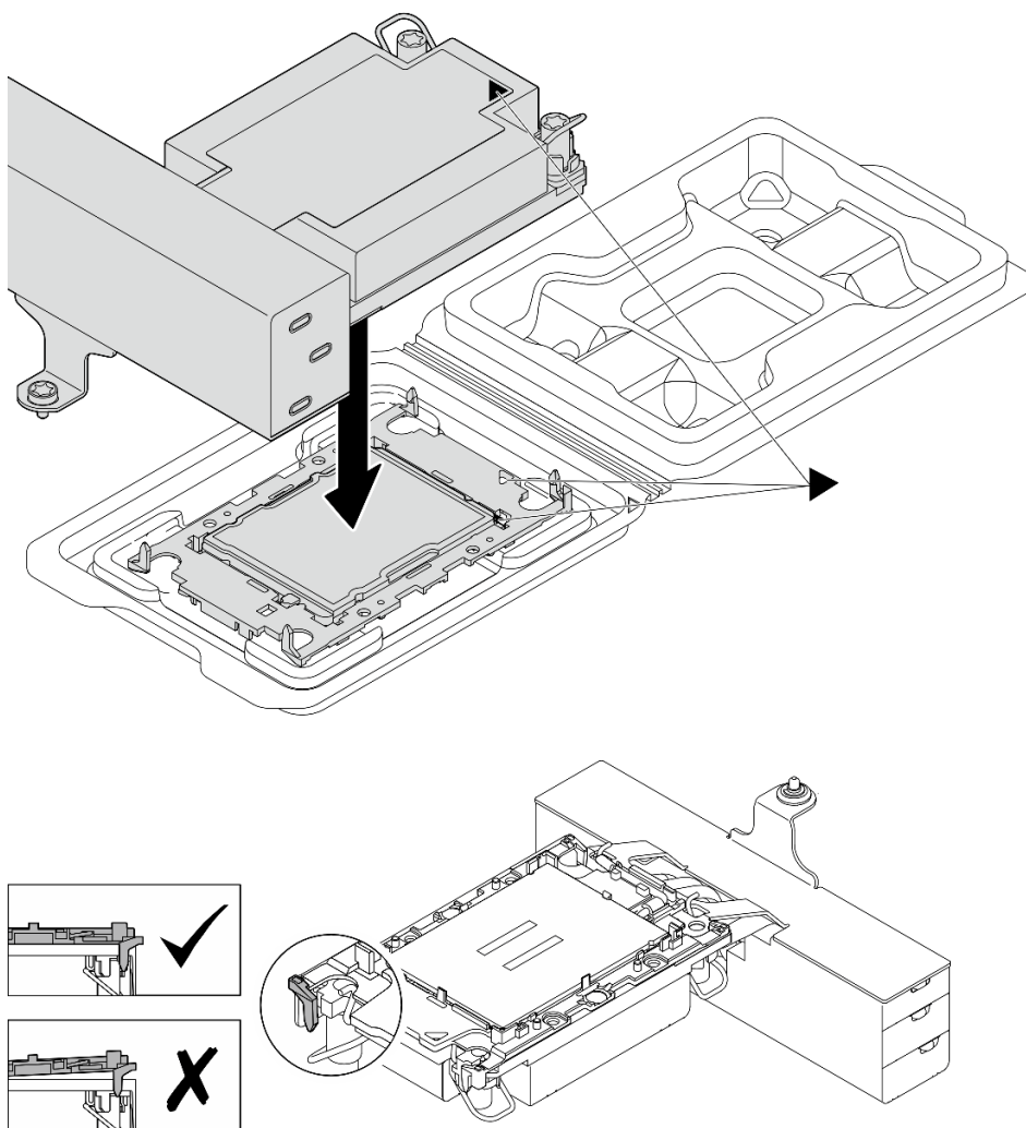
圖例 209. 將 PHM 和處理器裝到運送匣中
