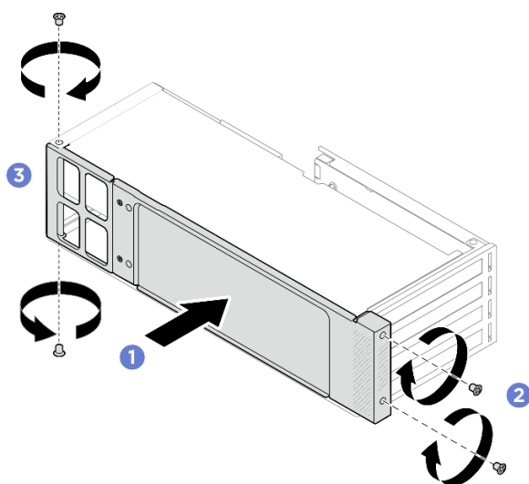
圖例 73. 安裝側面支撐托架
