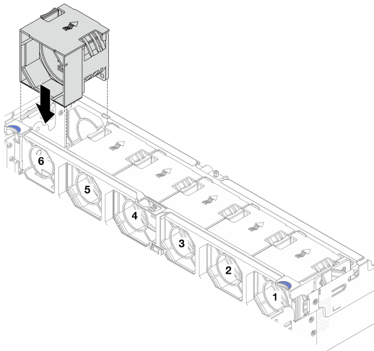
圖例 254. 安裝系統風扇
