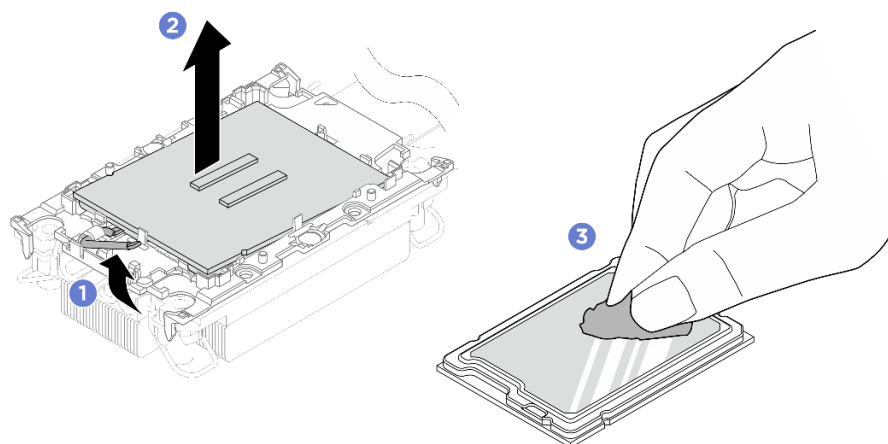
圖例 204. 將處理器與散熱槽和支架分開
