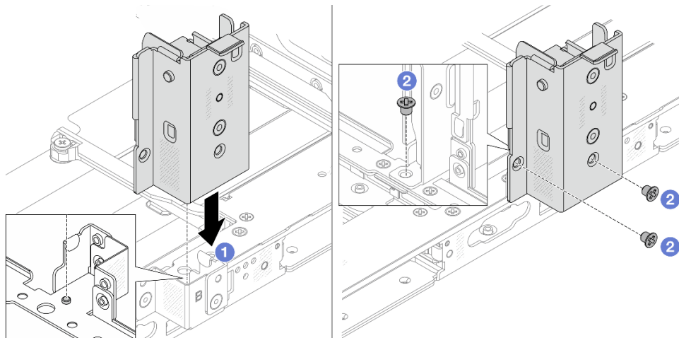
圖例 236. 安裝中間後壁托架
