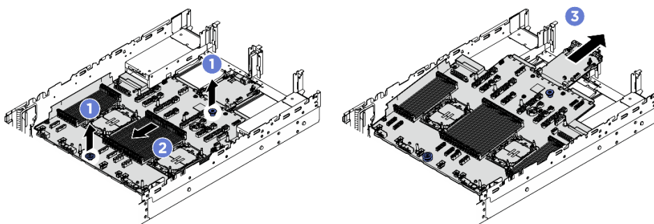
圖例 245. 卸下主機板組件
