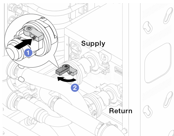
圖例 172. 開啟球閥
