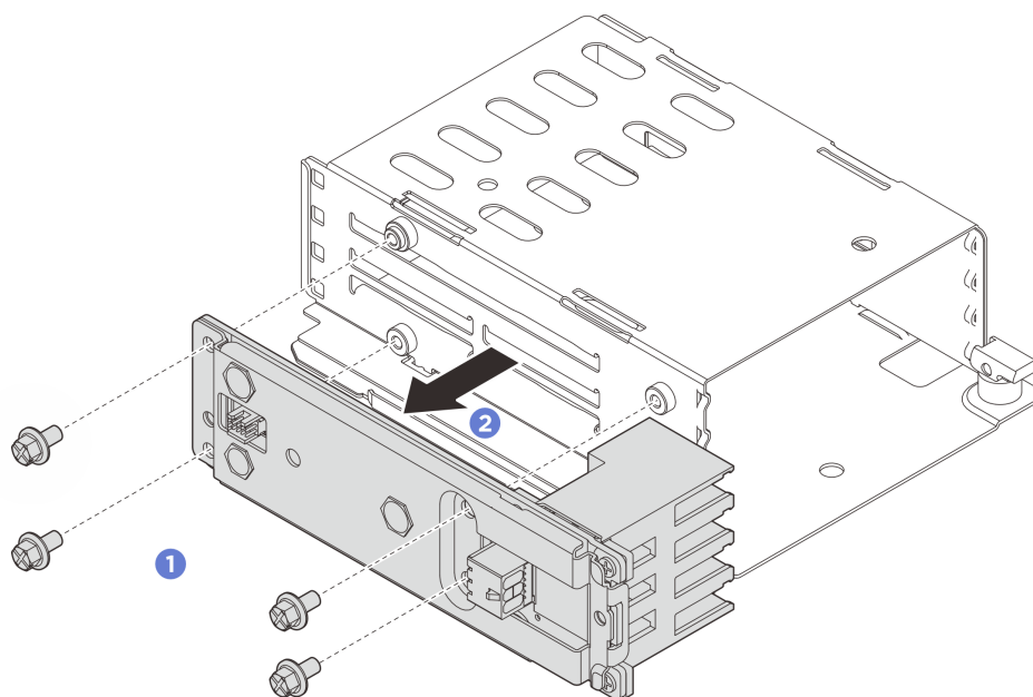
圖例 61. 卸下背板組件
