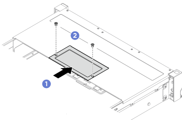
圖例 40. 安裝蓋板
