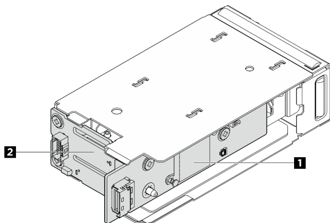
圖例 137. 前方 M.2 硬碟背板
