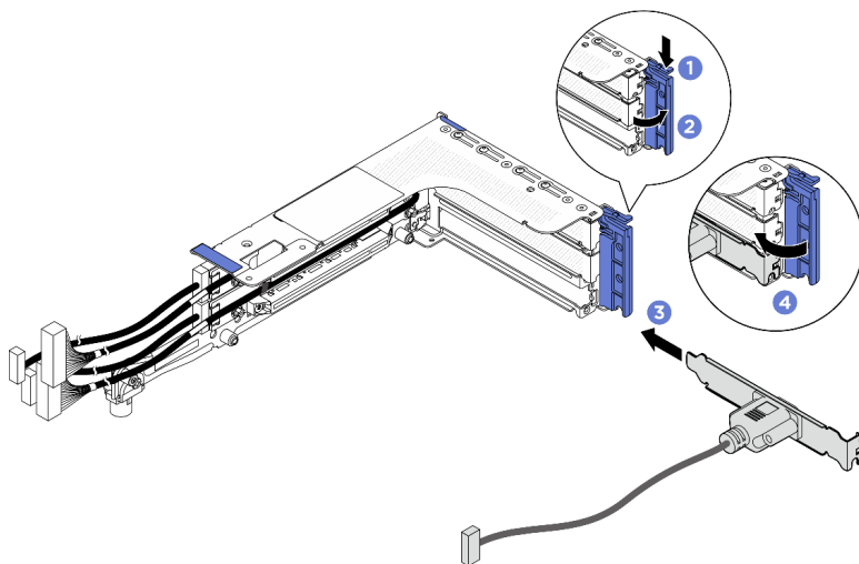
圖例 242. 安裝序列埠模組
