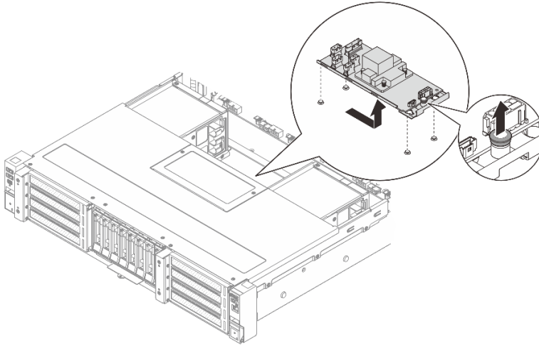
圖例 90. 卸下內部 CFF 配接卡
