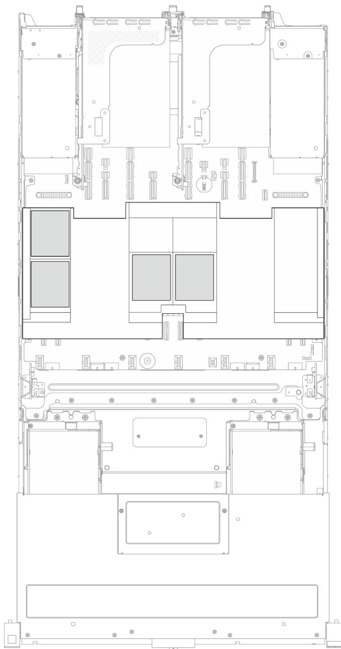
圖例 219. 空氣擋板上的 RAID 快閃記憶體電源模組位置
