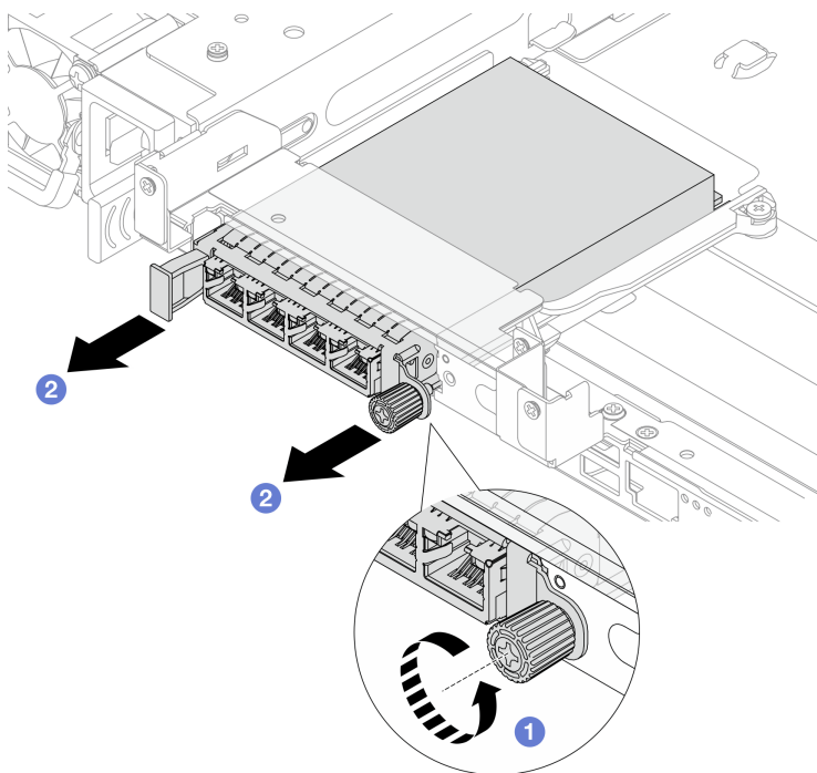
圖例 222. 卸下背面 OCP 模組
