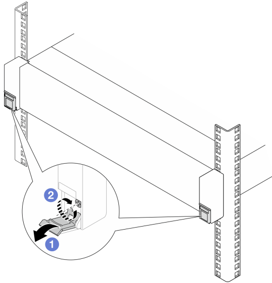
圖例 30. 將伺服器固定到機架正面
