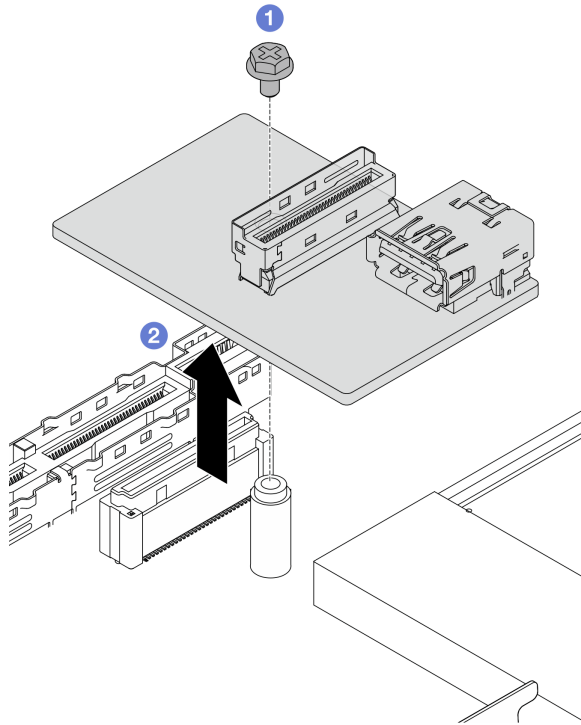
圖例 260. 卸下 USB I/O 板
