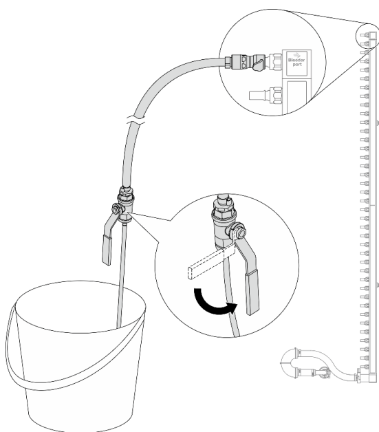
圖例 161. 開啟洩放閥門
