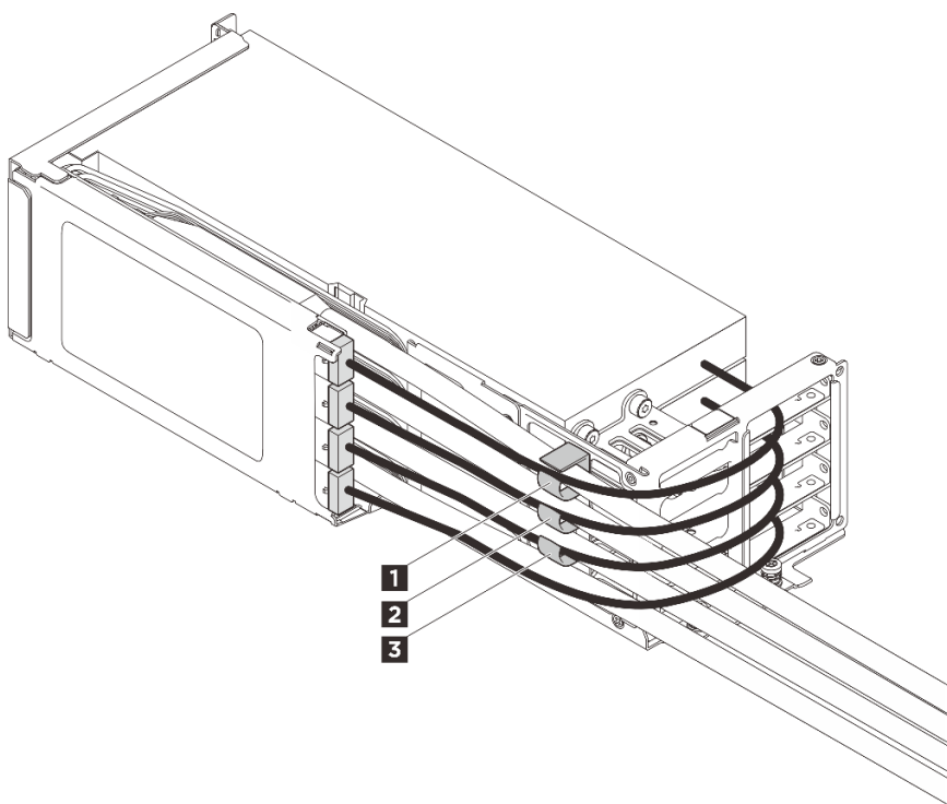
圖例 72. 正面擴充卡組件的纜線夾
