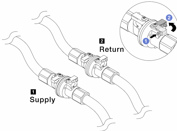
圖例 177. 關閉球閥
