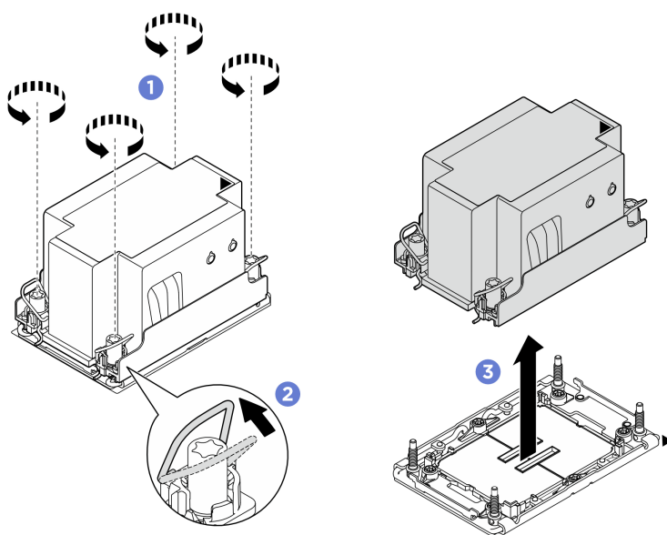
圖例 201. 卸下 2U 標準 PHM
