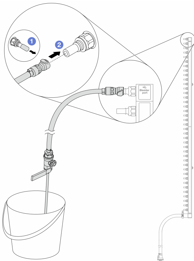
圖例 182. 在回流側安裝洩放套件
