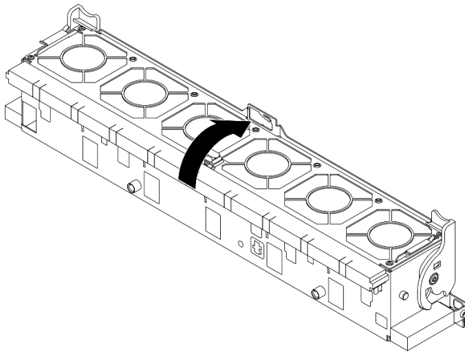
圖例 100. 旋轉風扇機盒
