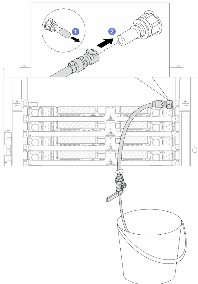
圖例 191. 在回流側安裝洩放套件
