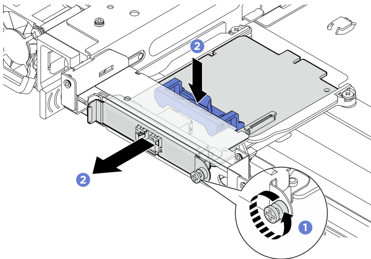
圖例 146. 卸下管理 NIC 配接卡
