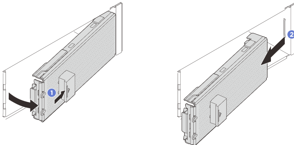
圖例 53. 卸下 E3.S 擋板
