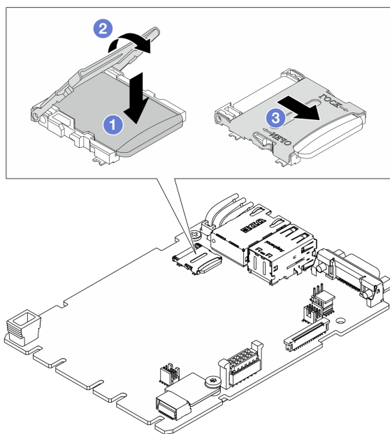
圖例 199. 安裝 MicroSD 卡
