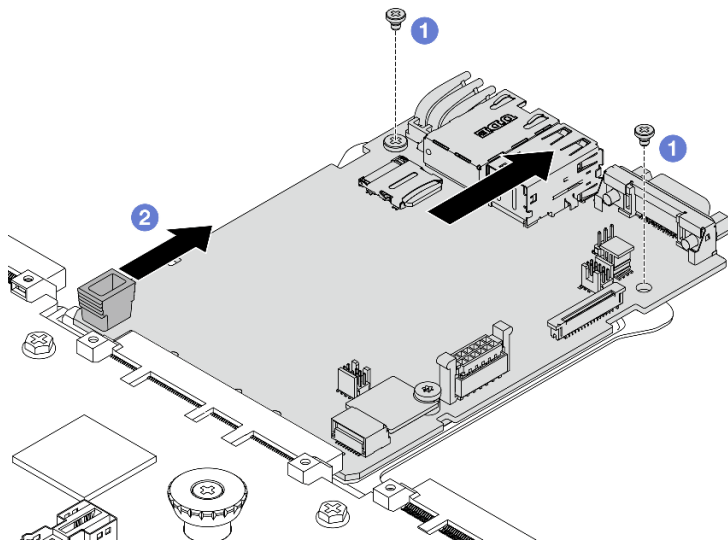
圖例 246. 將系統 I/O 板與處理器板分開
