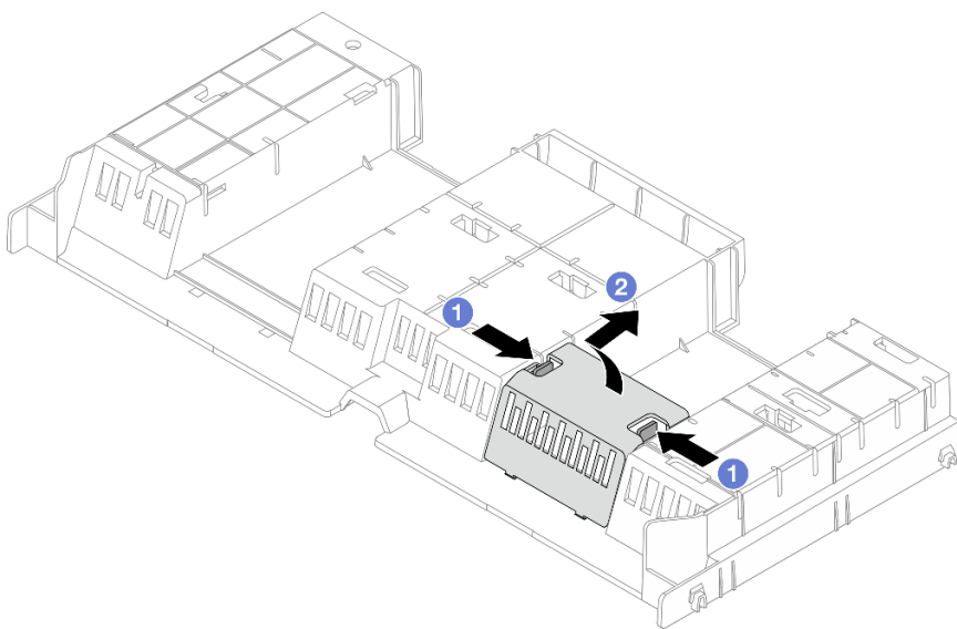
圖例 42. 卸下空氣擋板填充板
