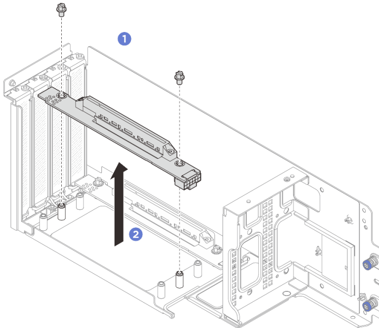
圖例 76. 卸下擴充卡
