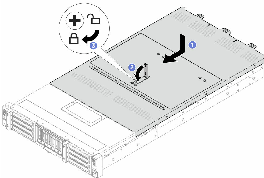
圖例 259. 安裝上蓋
