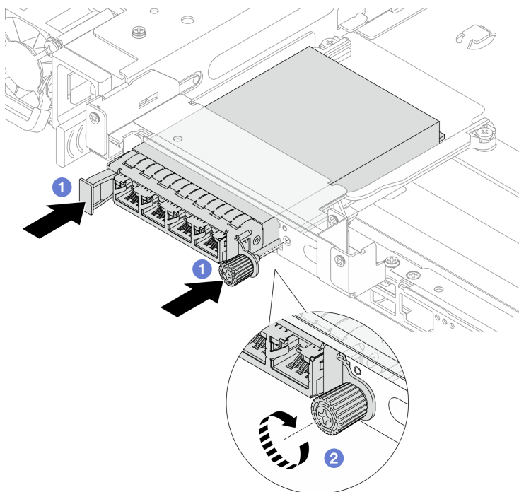
圖例 223. 安裝背面 OCP 模組
