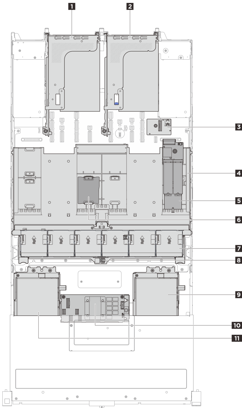
安裝空氣擋板後的俯視圖
