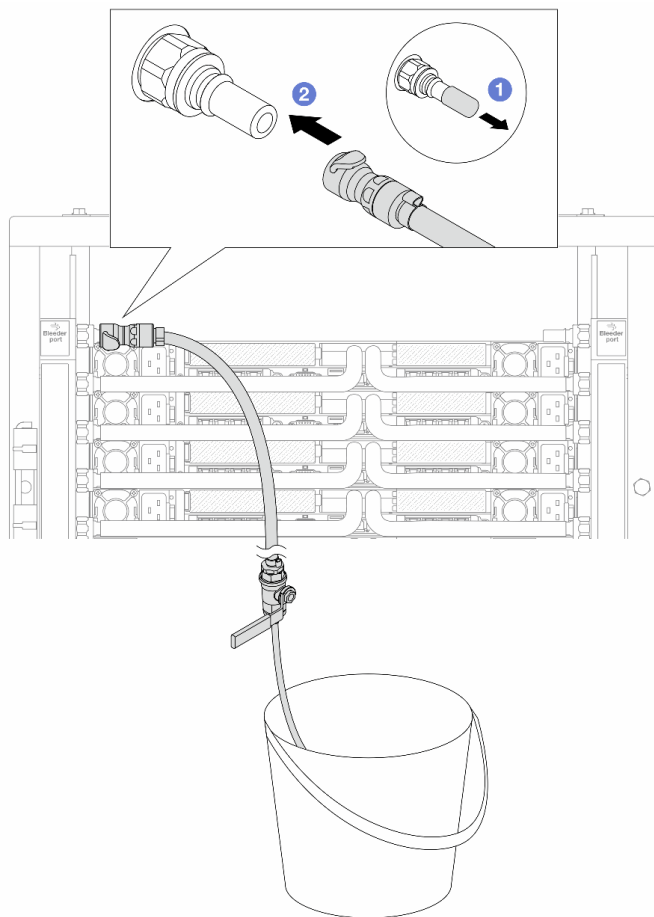
圖例 188. 安裝供應側的洩放套件
