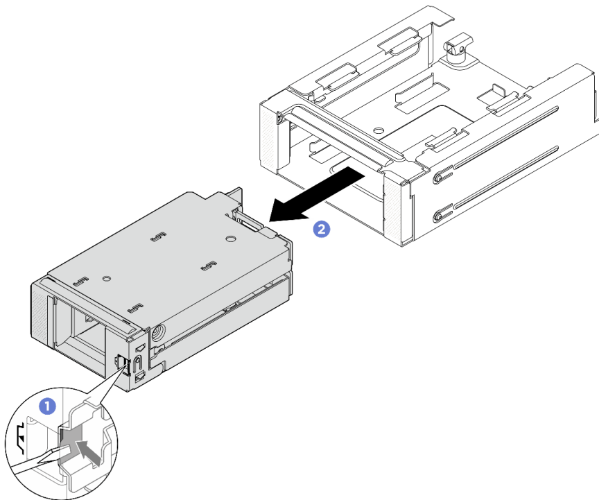
圖例 133. 從機架中卸下前方 M.2 框架
