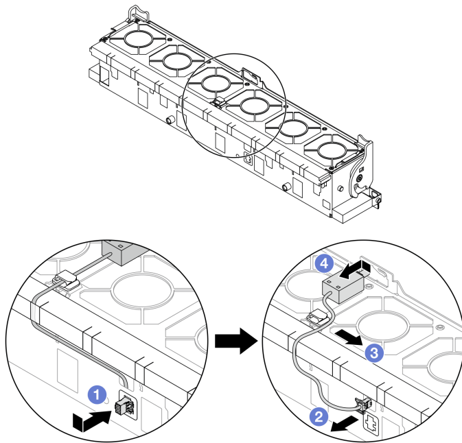
圖例 101. 卸下入侵開關
