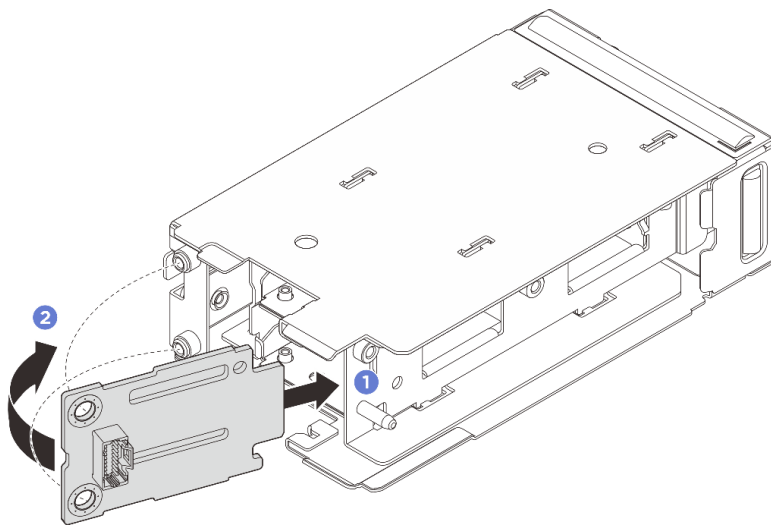
圖例 138. 安裝 M.2 開機背板
