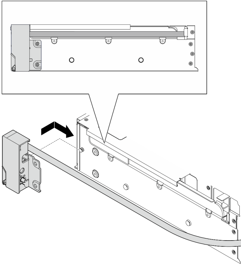
圖例 216. 安裝機架門鎖
