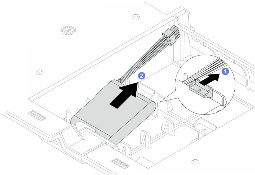
圖例 220. 從空氣擋板卸下 RAID 快閃記憶體電源模組
