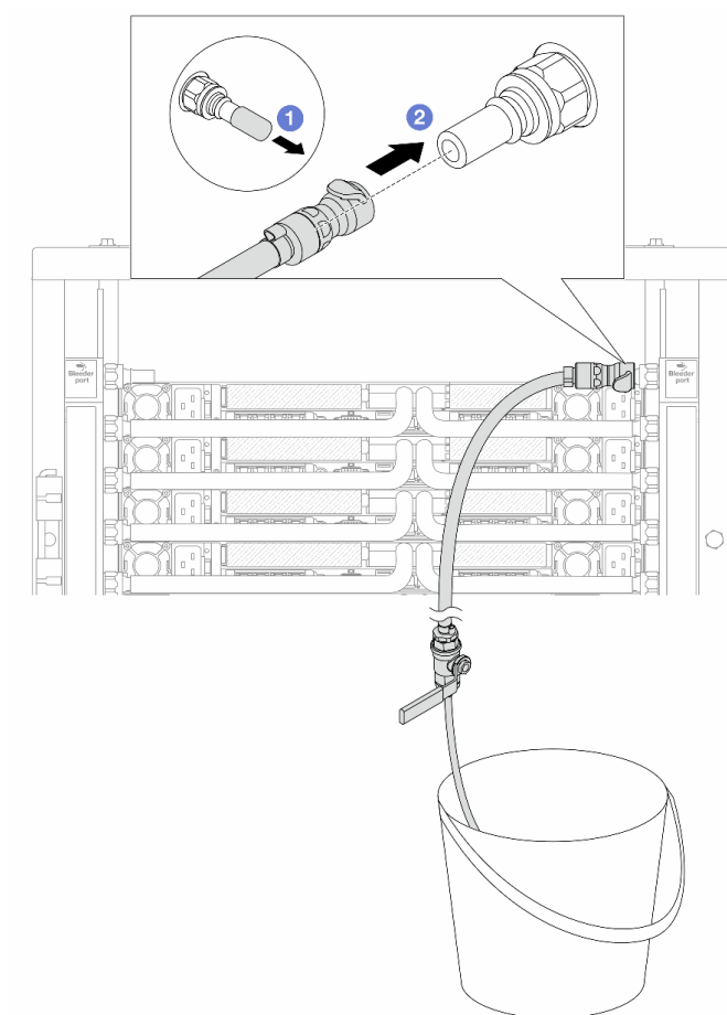
圖例 174. 在回流側安裝洩放套件
