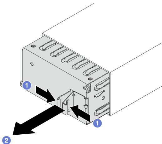
圖例 86. 卸下電源供應器填充板
