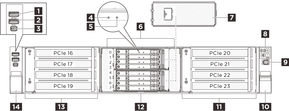
圖例 3. E3.S 硬碟配置的正面圖
