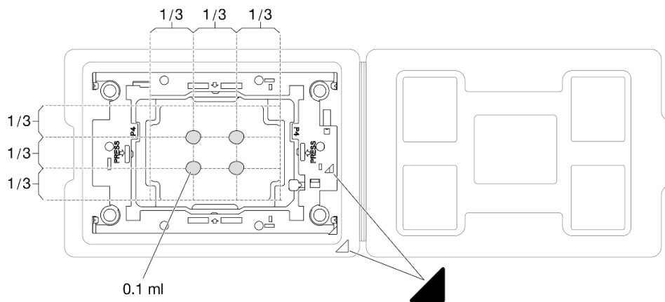
圖例 208. 運送匣中的處理器塗上散熱膏
