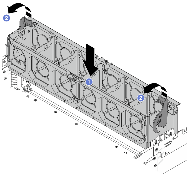
圖例 256. 安裝系統風扇機盒
