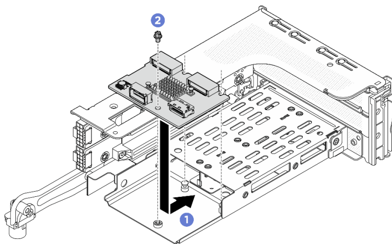
圖例 145. 將 M.2 背板安裝到 3FH M.2 擴充卡匣
