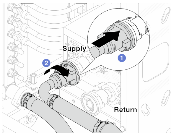
圖例 167. 連接球閥
