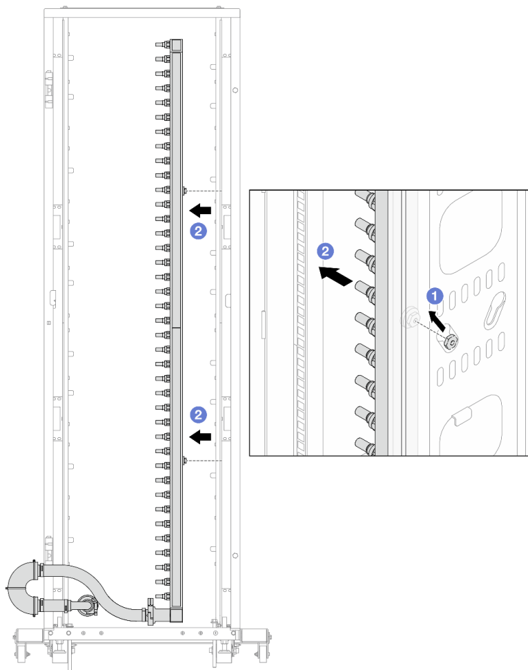
圖例 157. 卸下歧管
