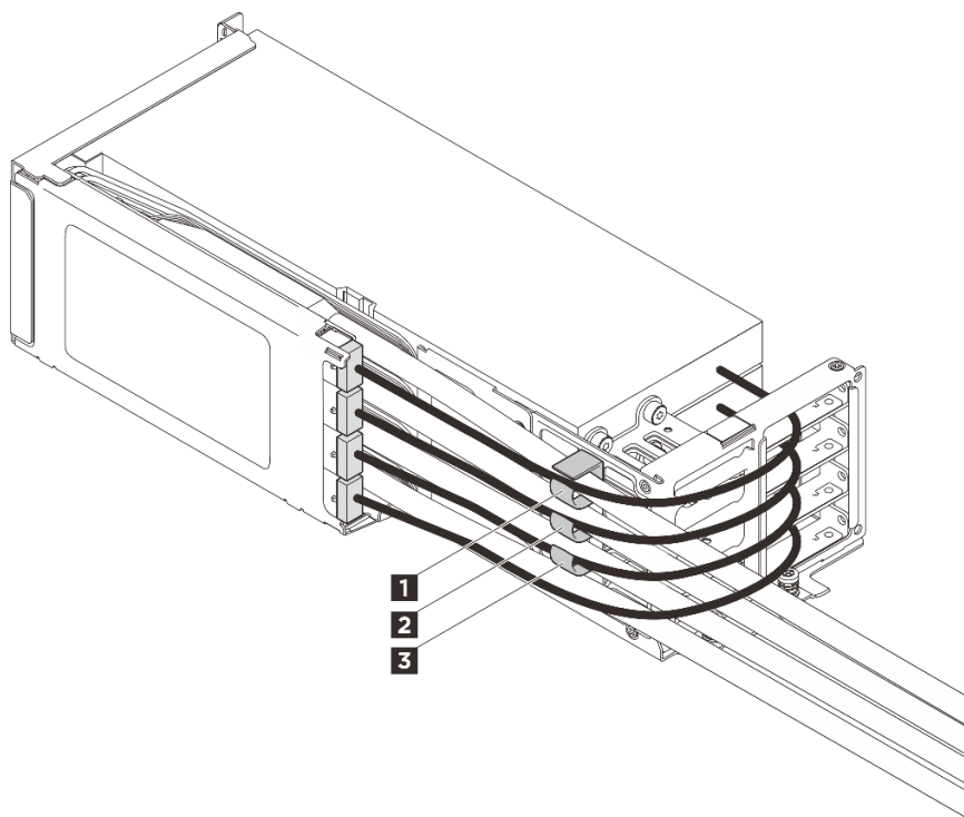
圖例 78. 正面擴充卡組件的纜線夾
