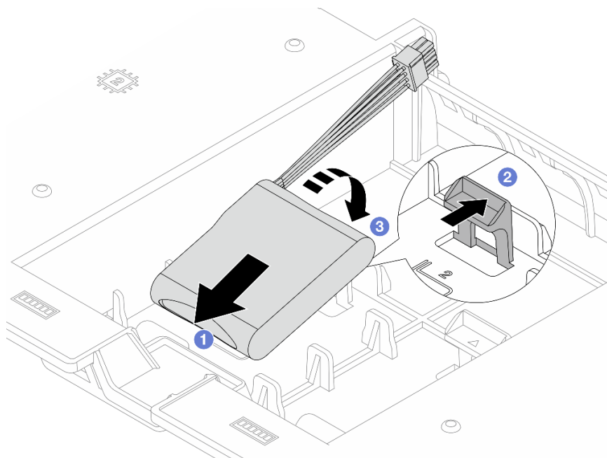
圖例 221. 將 RAID 快閃記憶體電源模組安裝在空氣擋板上
