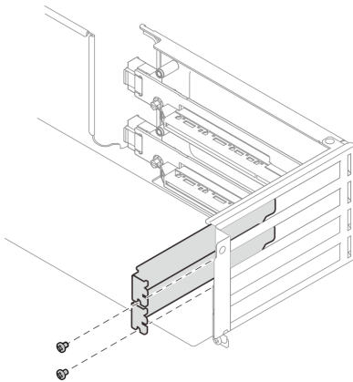
圖例 69. PCIe 插槽填充板
