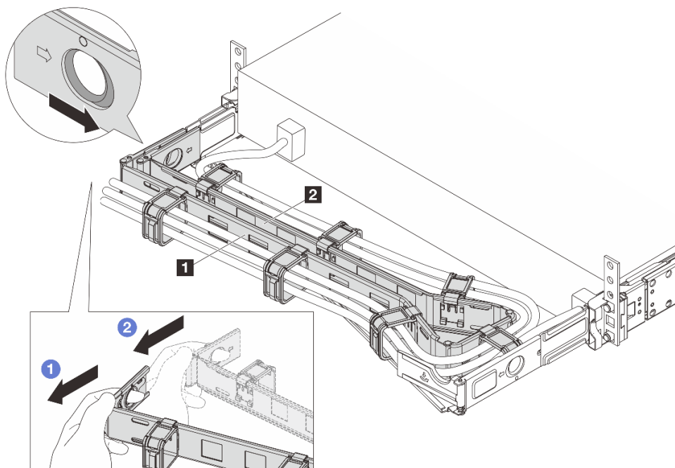
圖例 82. 卸下左側
