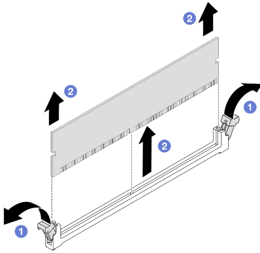
圖例 196. 卸下記憶體模組
