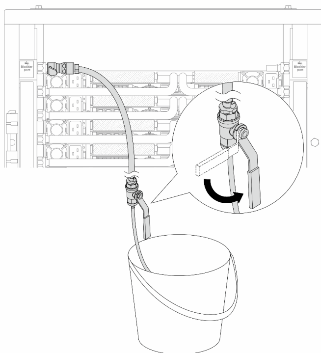
圖例 190. 開啟供應側的洩放閥門
