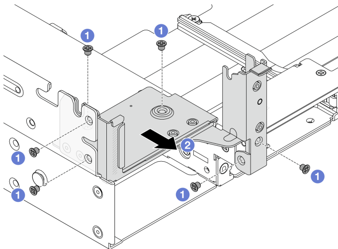
圖例 232. 卸下左側後壁托架
