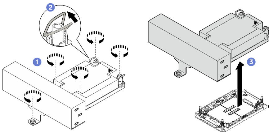
圖例 202. 卸下 1U T 形效能 PHM
