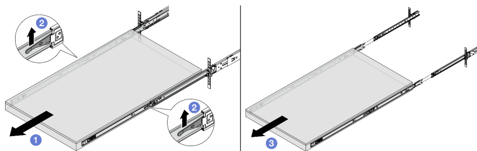
圖例 23. 拉出伺服器
