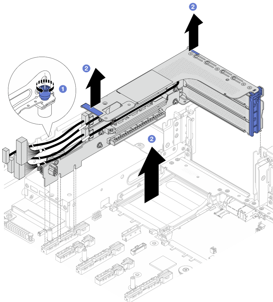
圖例 226. 卸下 3FH 擴充卡組件
