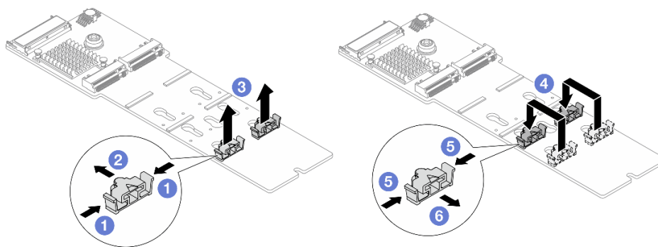
圖例 93. 調整 M.2 固定器
