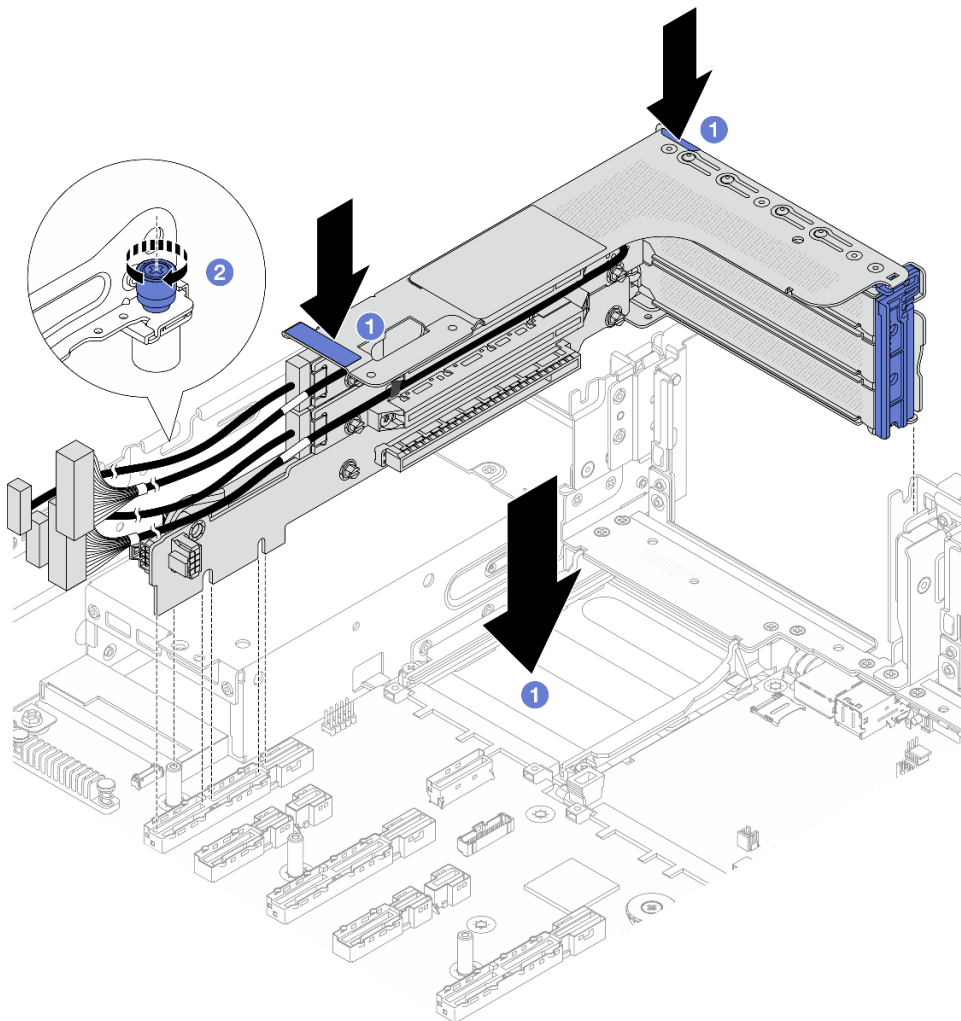
圖例 231. 安裝 3FH 擴充卡組件
