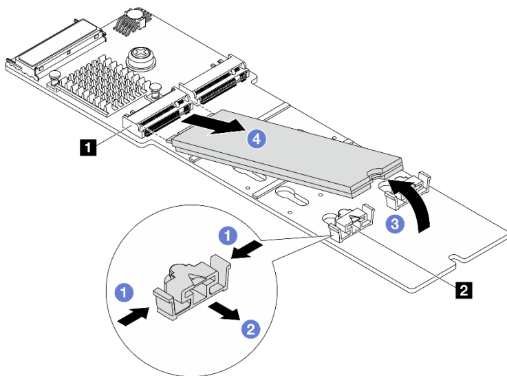
圖例 92. 卸下 M.2 硬碟
