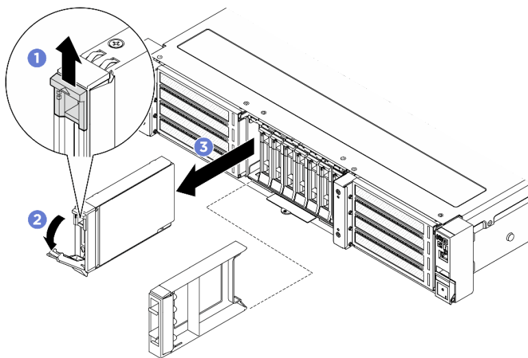
圖例 32. 卸下 2.5 吋熱抽換硬碟
