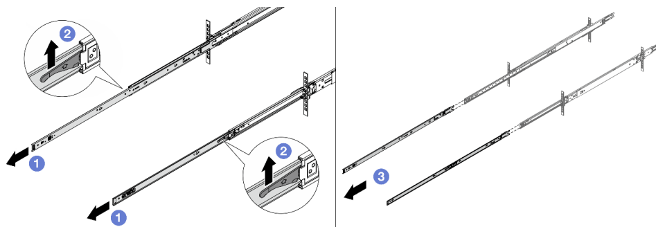
圖例 25. 拉出滑軌
