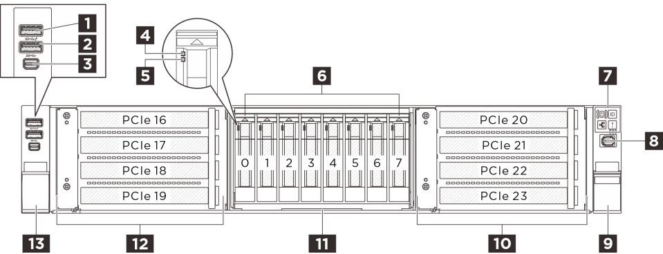
圖例 2. 2.5 吋硬碟配置的正面圖
