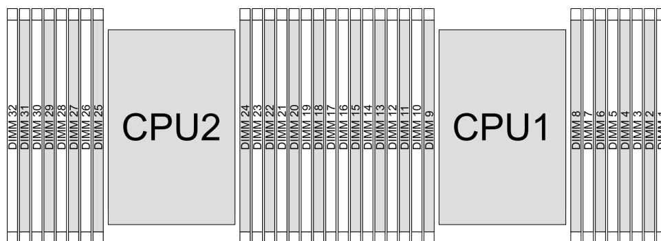
圖例 15. 處理器板上的記憶體模組插槽
