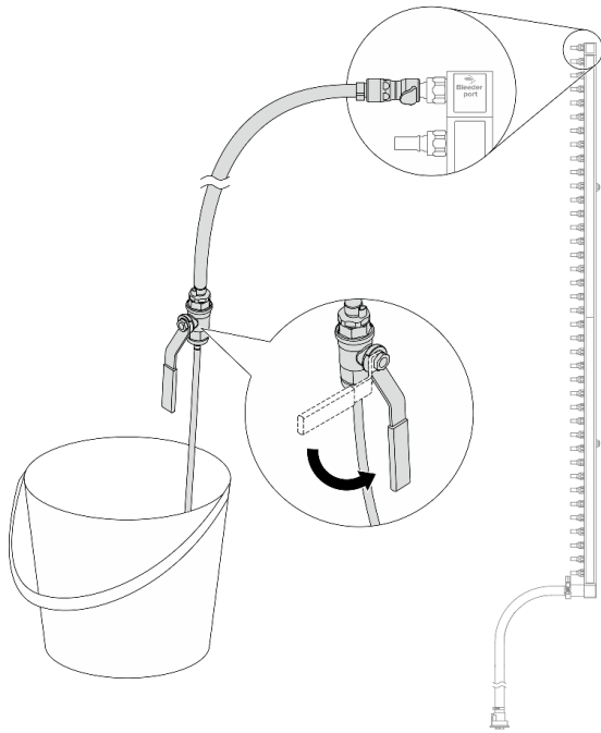
圖例 183. 開啟洩放閥門
