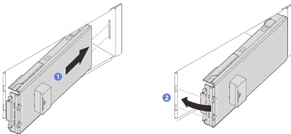
圖例 58. 安裝 E3.S 擋板
