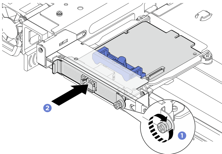
圖例 147. 安裝管理 NIC 配接卡
