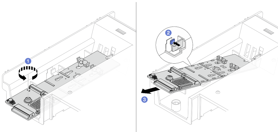
圖例 97. 從空氣擋板卸下 M.2 背板
