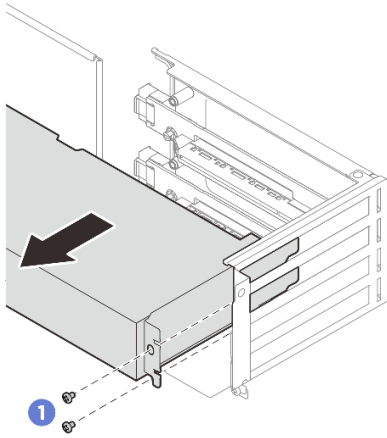
圖例 68. 卸下 PCIe 配接卡
