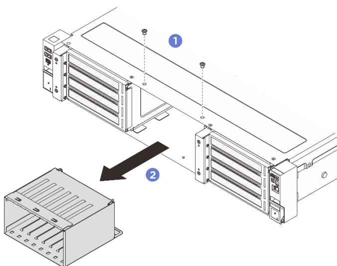
圖例 37. 卸下 2.5 吋框架
