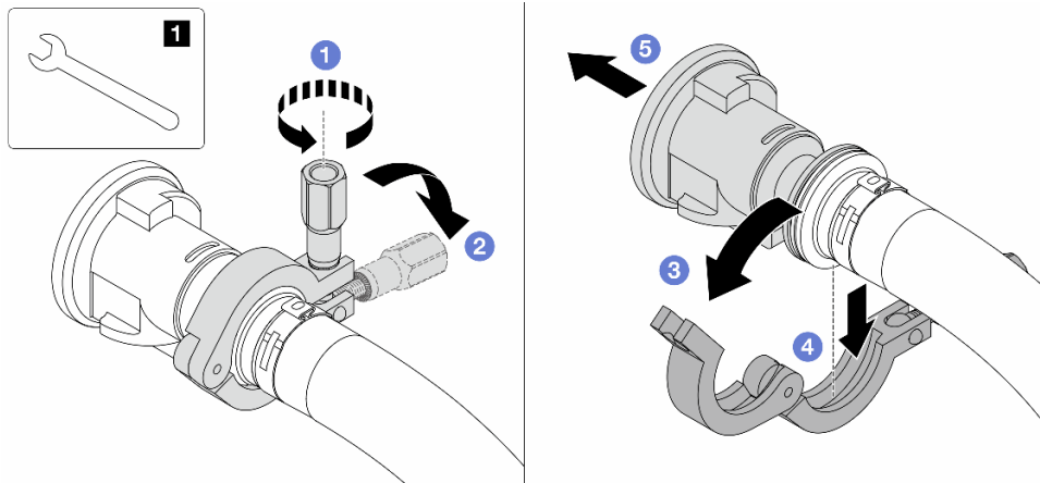
圖例 164. 分開球閥
