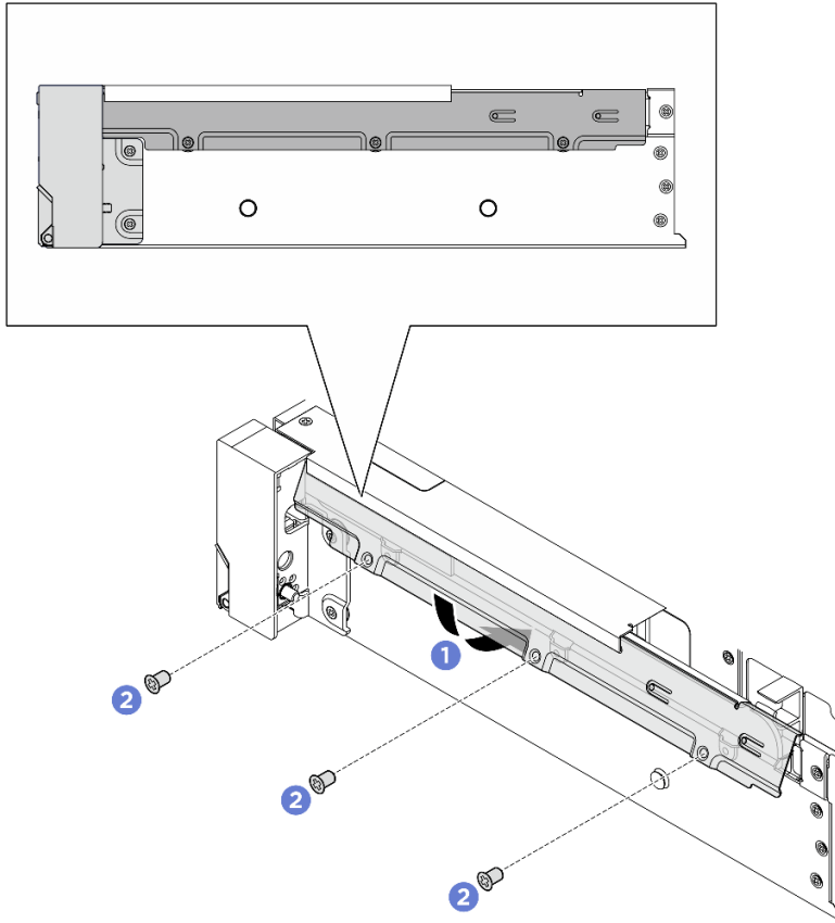
圖例 218. 安裝纜線固定夾
