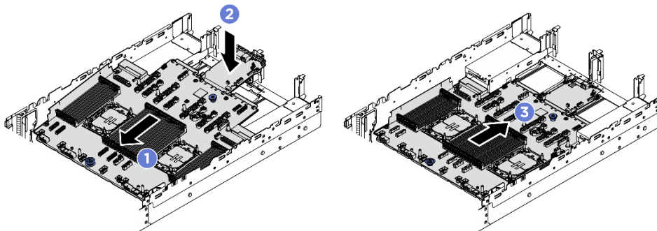
圖例 248. 安裝主機板組件
