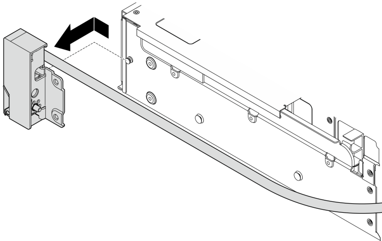
圖例 215. 卸下機架門鎖
