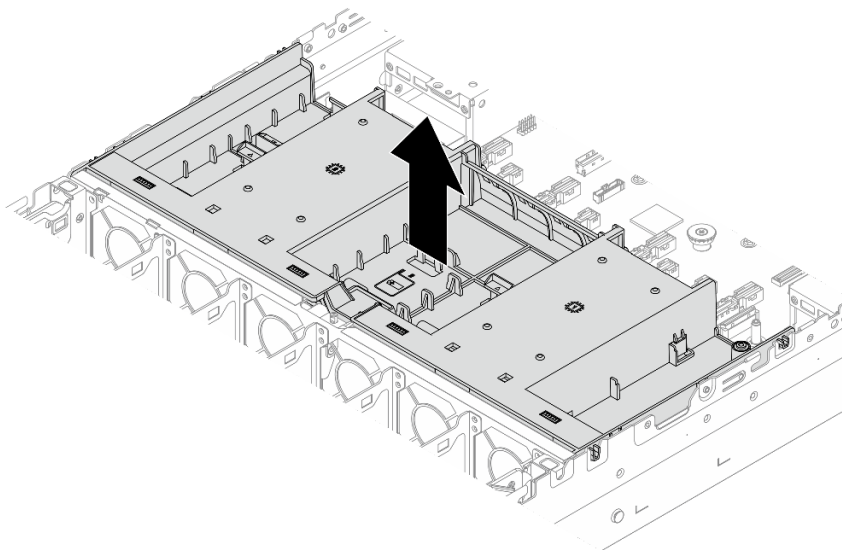
圖例 41. 卸下空氣擋板
