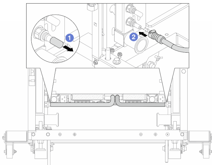
圖例 186. 安裝快速連接插件
