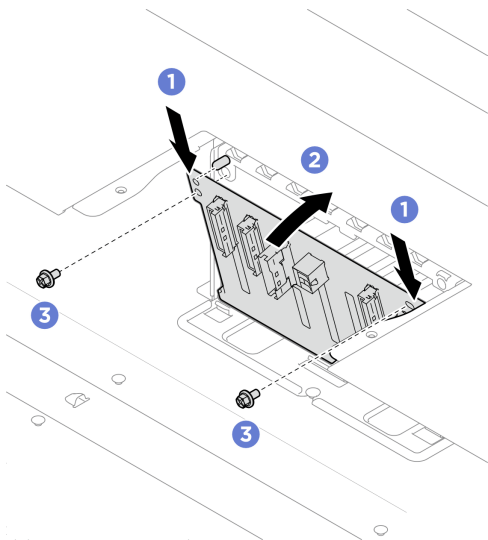
圖例 39. 安裝 2.5 吋硬碟背板
