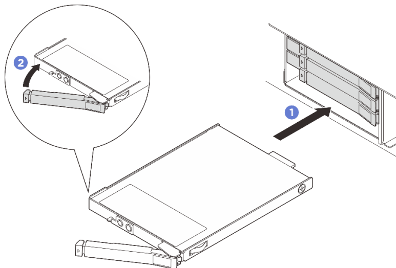
圖例 55. 安裝 E3.S 熱抽換硬碟
