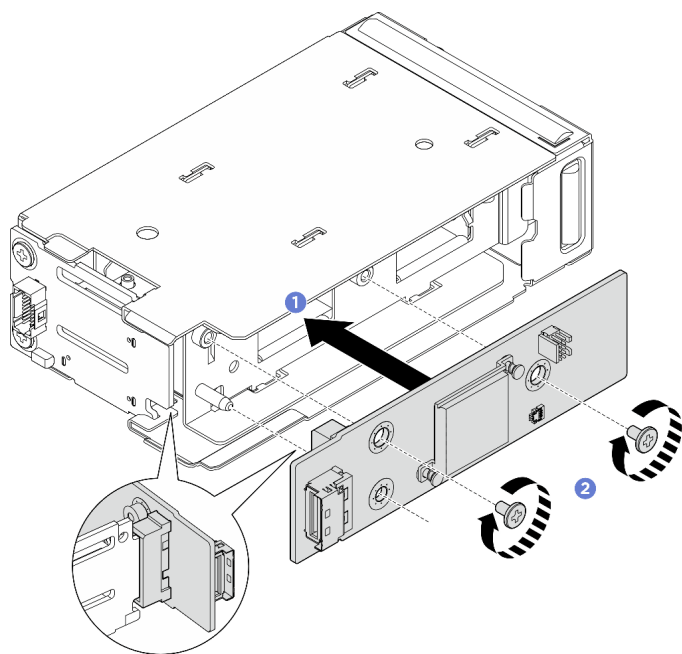
圖例 140. 安裝前方 M.2 控制器板
