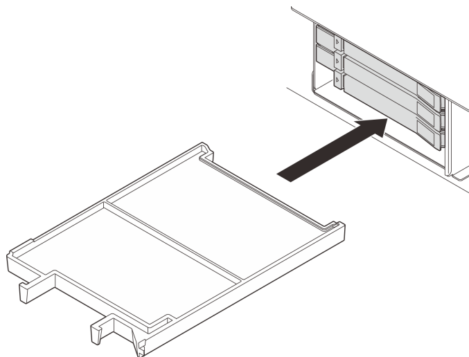
圖例 56. 安裝機槽填充板
