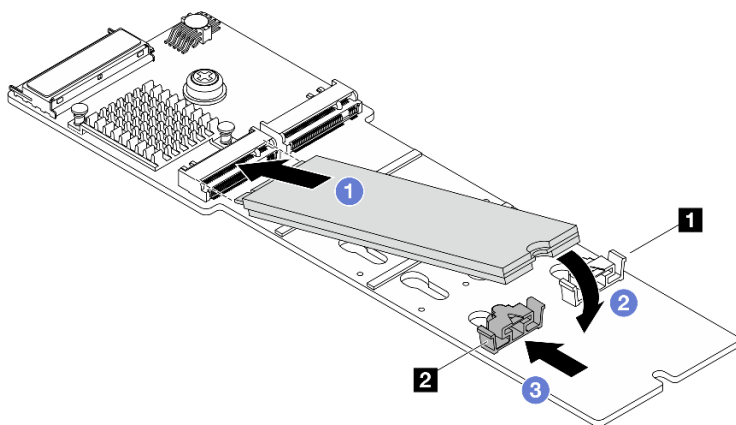
圖例 95. 安裝 M.2 硬碟
