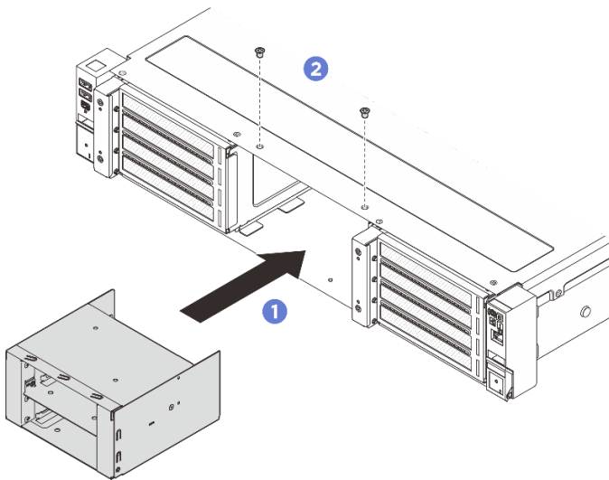
圖例 63. 安裝 E3.S 框架
