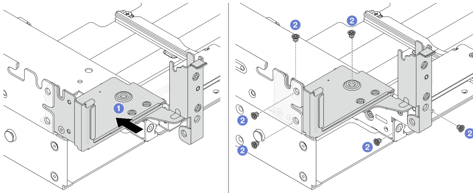
圖例 235. 安裝左側後壁托架
