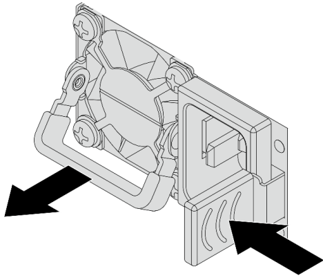
圖例 83. 卸下熱抽換電源供應器
