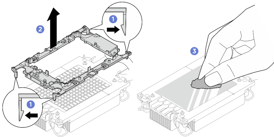
圖例 205. 將處理器支架與散熱槽分開
