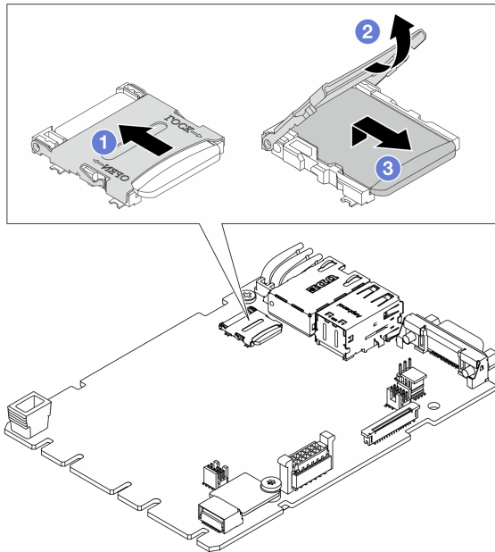
圖例 198. 卸下 MicroSD 卡
