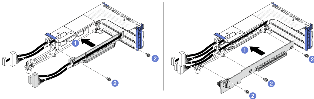
圖例 229. 在 3FH 擴充卡匣上安裝擴充卡
