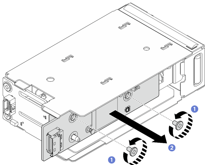
圖例 134. 卸下前方 M.2 控制器板
