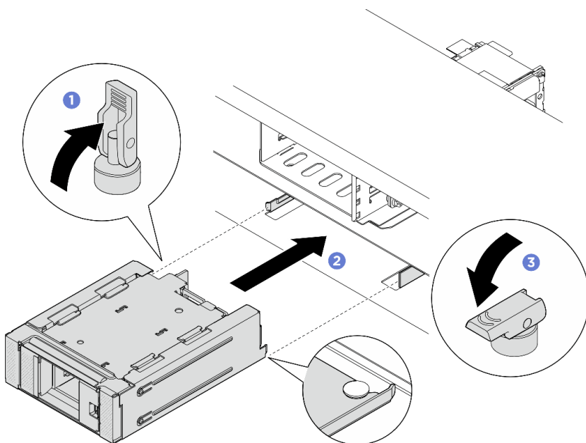
圖例 142. 安裝前方 M.2 框架及其機架
