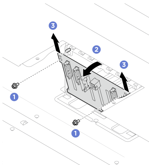
圖例 36. 卸下 2.5 吋硬碟背板
