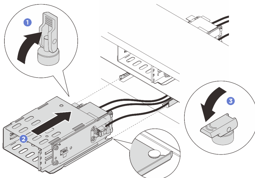
圖例 65. 安裝 E3.S 1T 框架
