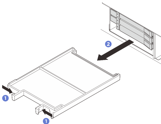
圖例 54. 卸下機槽填充板
