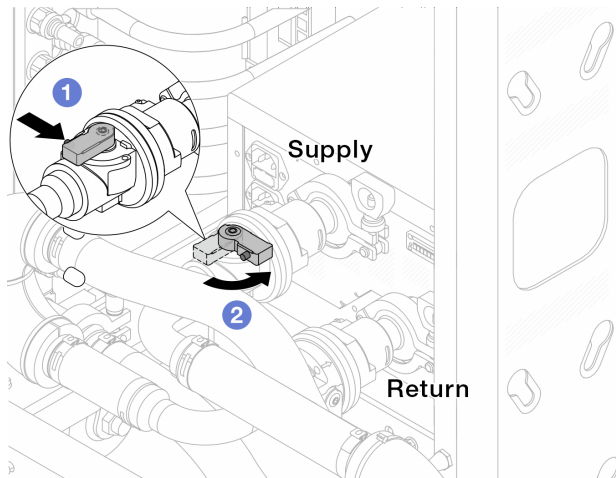
圖例 154. 關閉球閥
