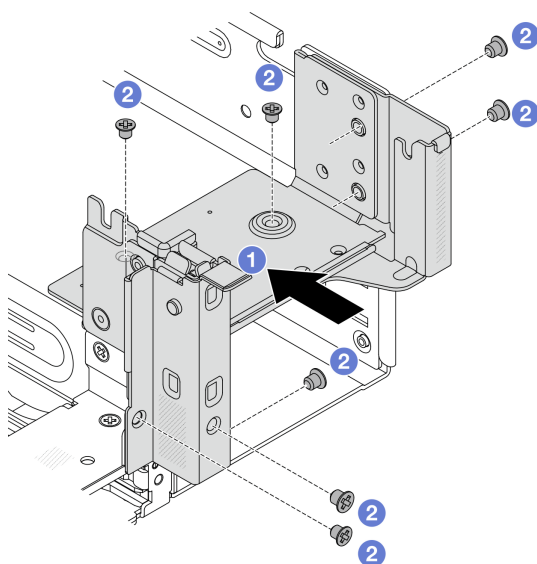
圖例 237. 安裝右側後壁托架
