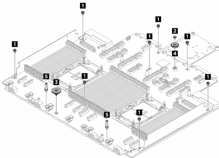
圖例 278. 拆卸主機板組件
