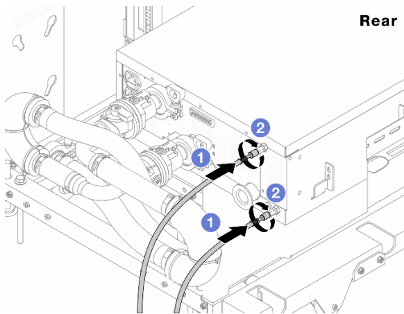
圖例 169. CDU 的背面
