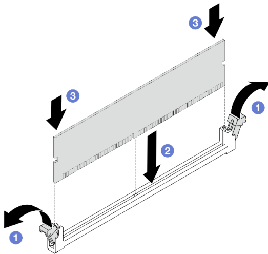
圖例 197. 安裝記憶體模組
