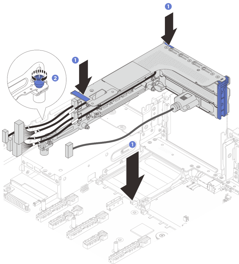
圖例 243. 安裝擴充卡組件
