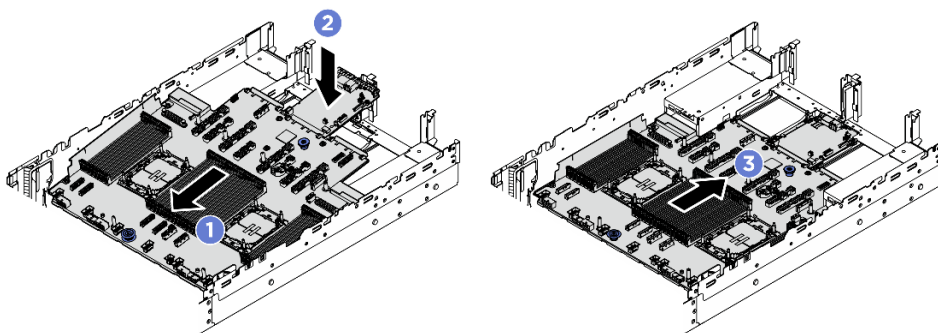
圖例 252. 安裝主機板組件
