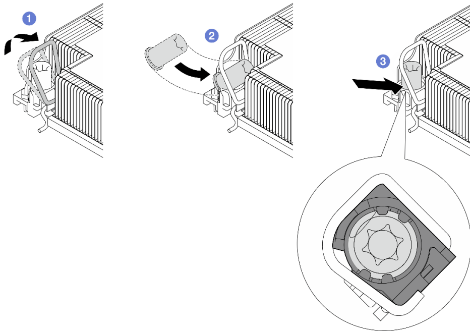
圖例 80. 將 Torx T30 螺帽安裝到散熱槽
