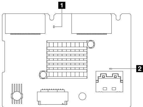
圖例 270. 背面 M.2 背板 LED
