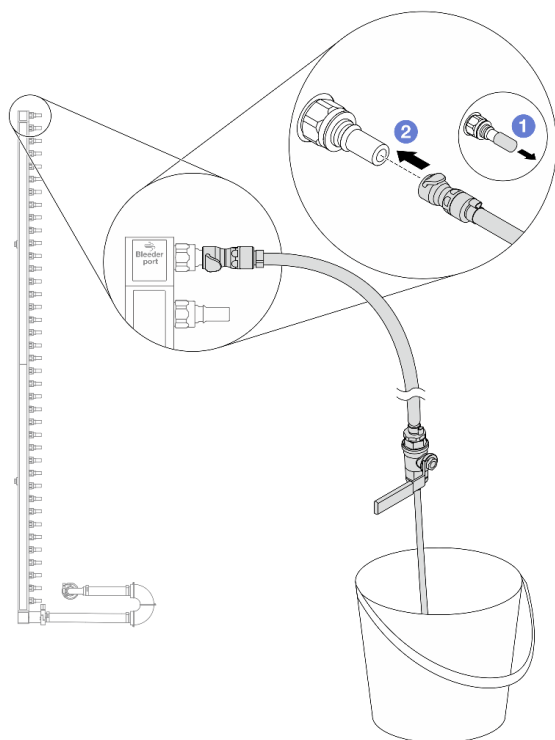
圖例 158. 安裝供應側的洩放套件
