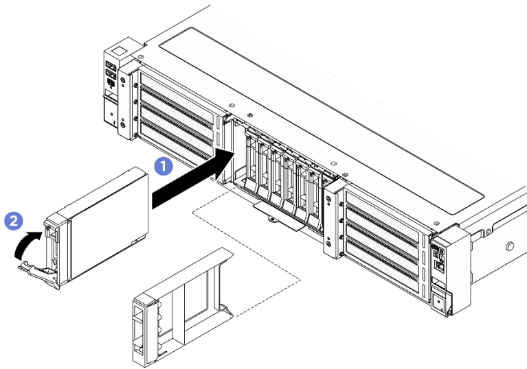
圖例 34. 安裝 2.5 吋熱抽換硬碟
