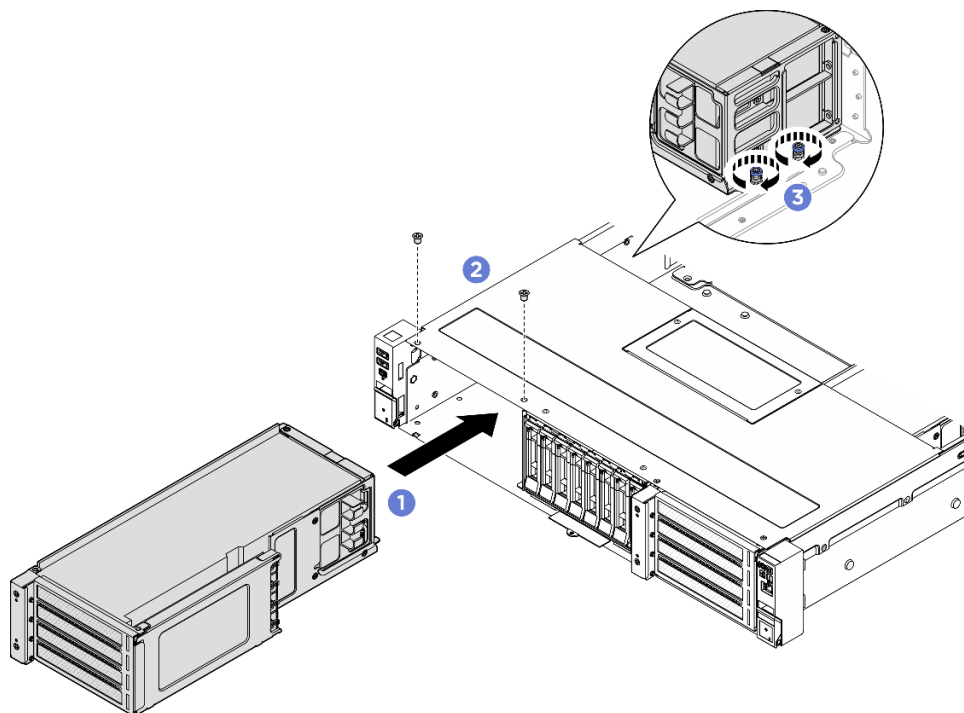
圖例 74. 安裝正面擴充卡組件
