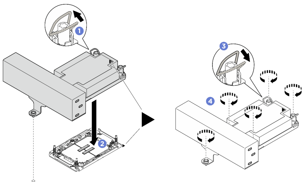
圖例 212. 安裝 1U T 形效能 PHM
