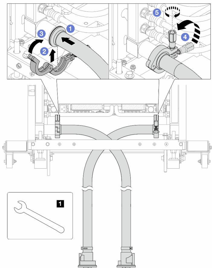
圖例 187. 安裝水管套件
