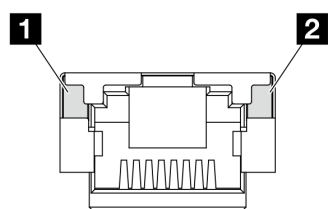
圖例 268. XCC 系統管理埠 (10/100/1000 Mbps RJ-45) 上的 LED
