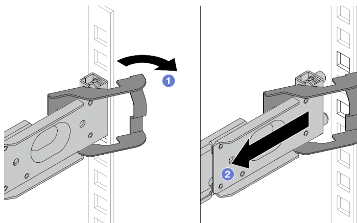
圖例 18. 從後方卸下滑軌
