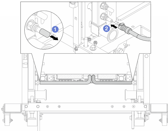
圖例 170. 安裝快速連接插件
