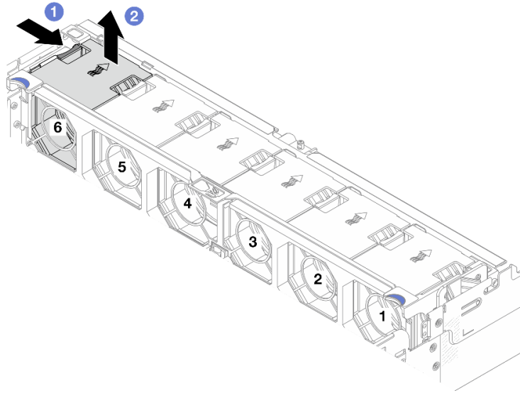
圖例 253. 卸下系統風扇
