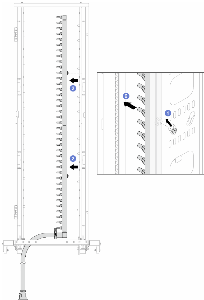
圖例 179. 卸下歧管
