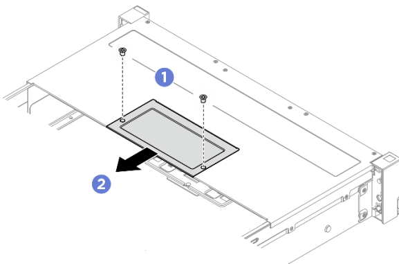
圖例 89. 卸下蓋板
