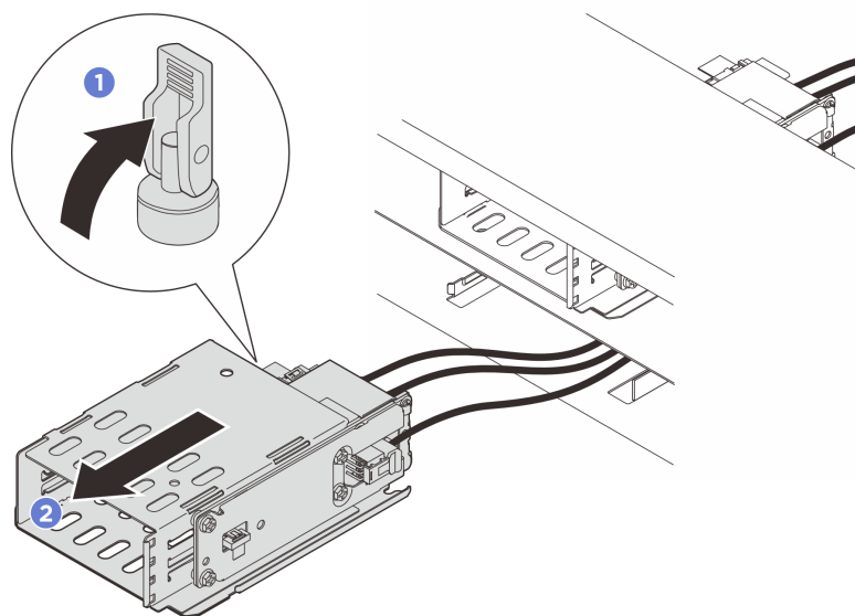
圖例 60. 卸下 E3.S 1T 框架
