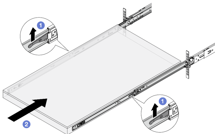
圖例 29. 鎖定滑軌，並將伺服器滑入
