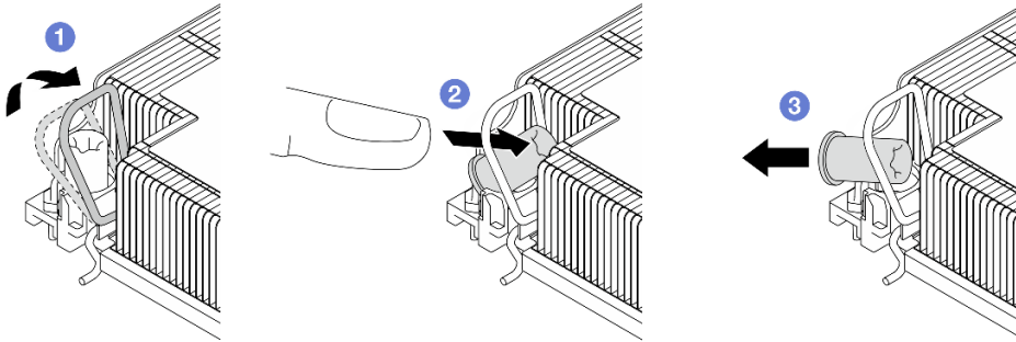
圖例 79. 從散熱槽卸下 Torx T30 螺帽
