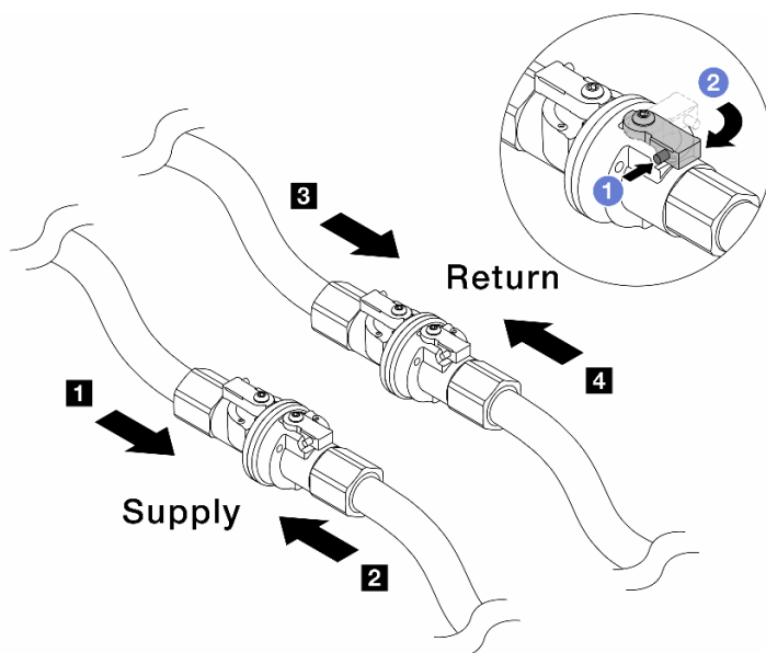
圖例 195. 開啟球閥
