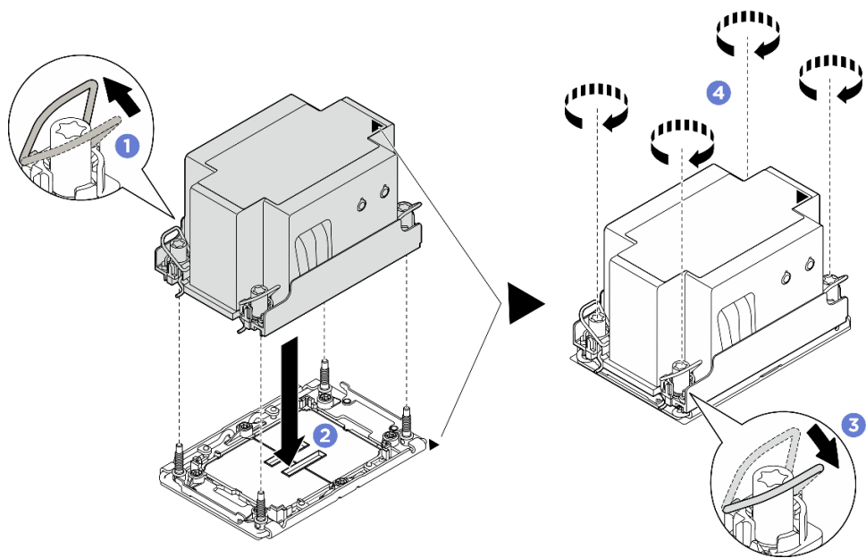
圖例 211. 安裝 2U 標準 PHM
