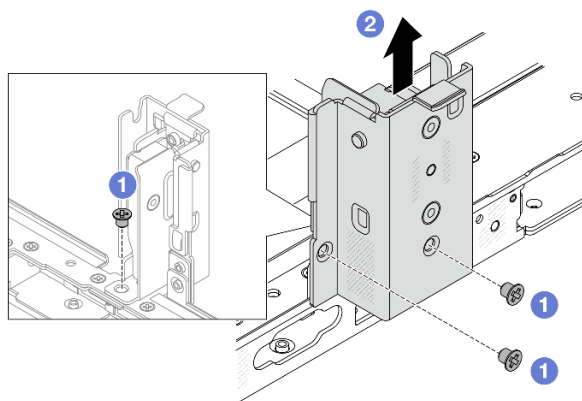
圖例 233. 卸下中間後壁托架
