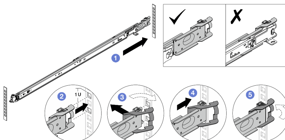
圖例 19. 安裝後方安裝插腳
