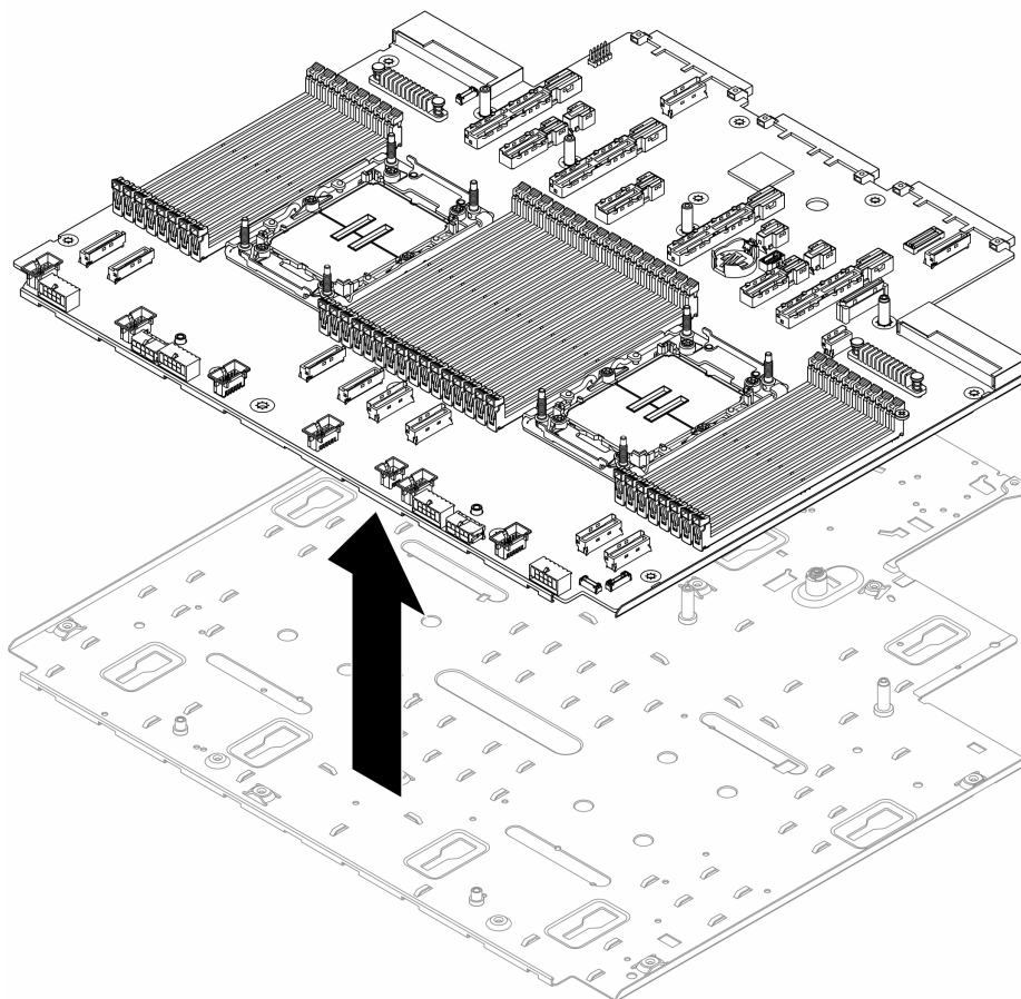
圖例 280. 分開處理器板
