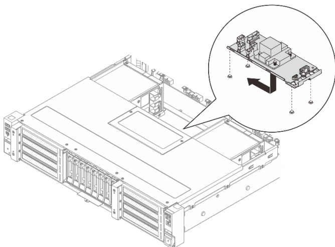
圖例 91. 安裝內部 CFF 配接卡
