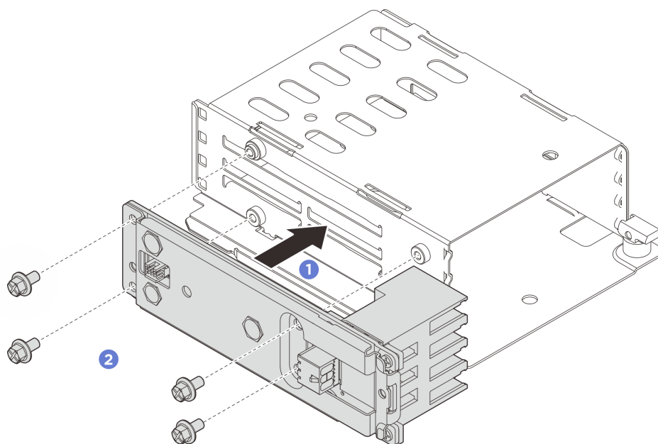
圖例 64. 安裝背板組件
