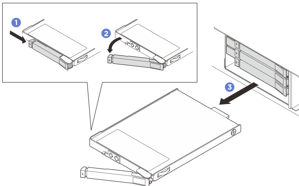
圖例 52. 卸下 E3.S 熱抽換硬碟
