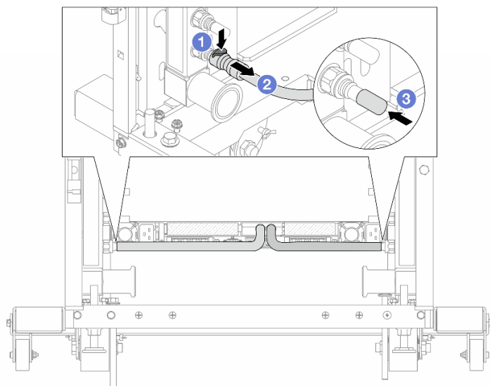
圖例 178. 移除 quick connect 插頭
