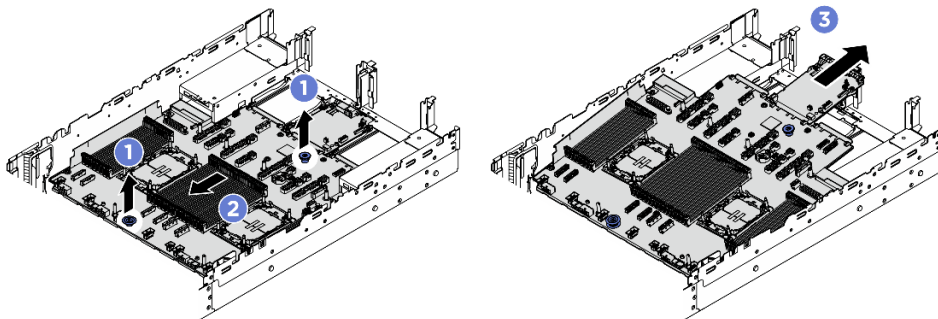
圖例 249. 卸下主機板組件
