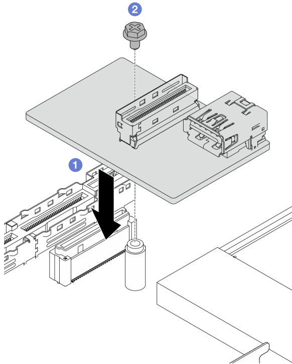
圖例 261. 安裝 USB I/O 板
