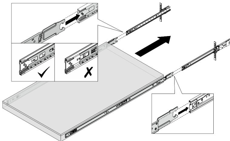
圖例 28. 交互鎖定滑軌
