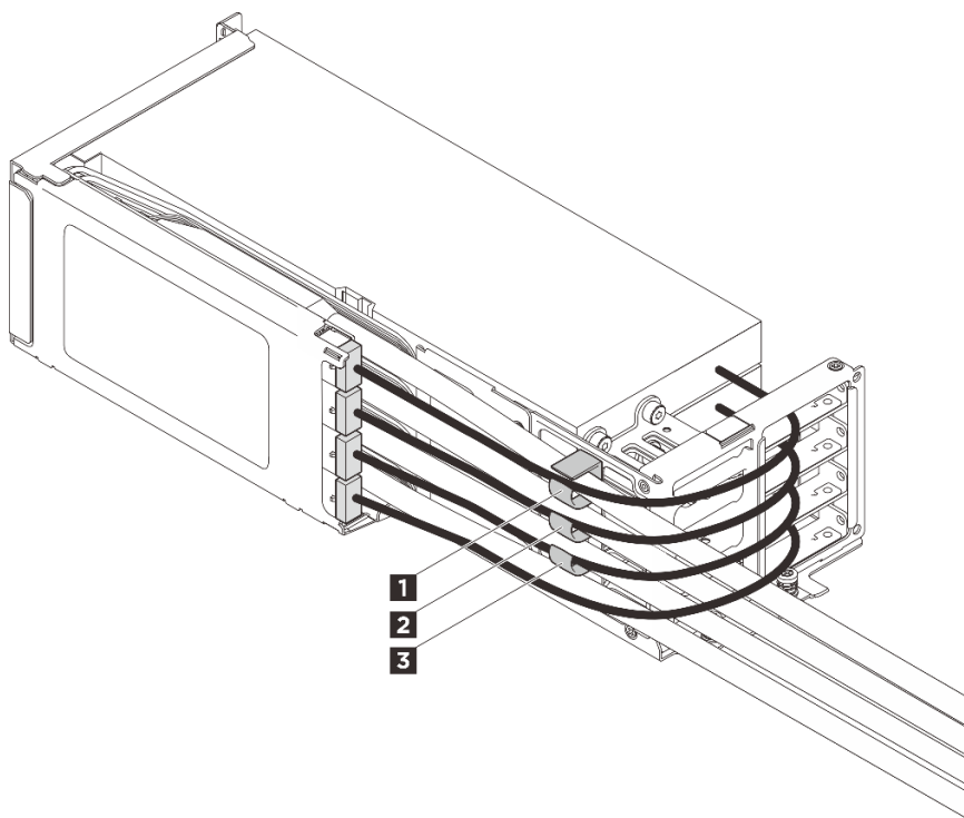
圖例 75. 正面擴充卡組件的纜線夾
