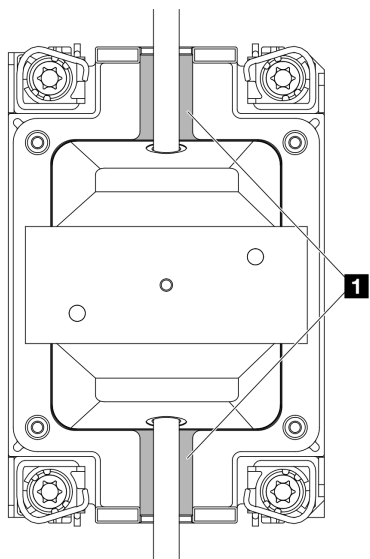
圖例 276. 易發生洩漏的區域
