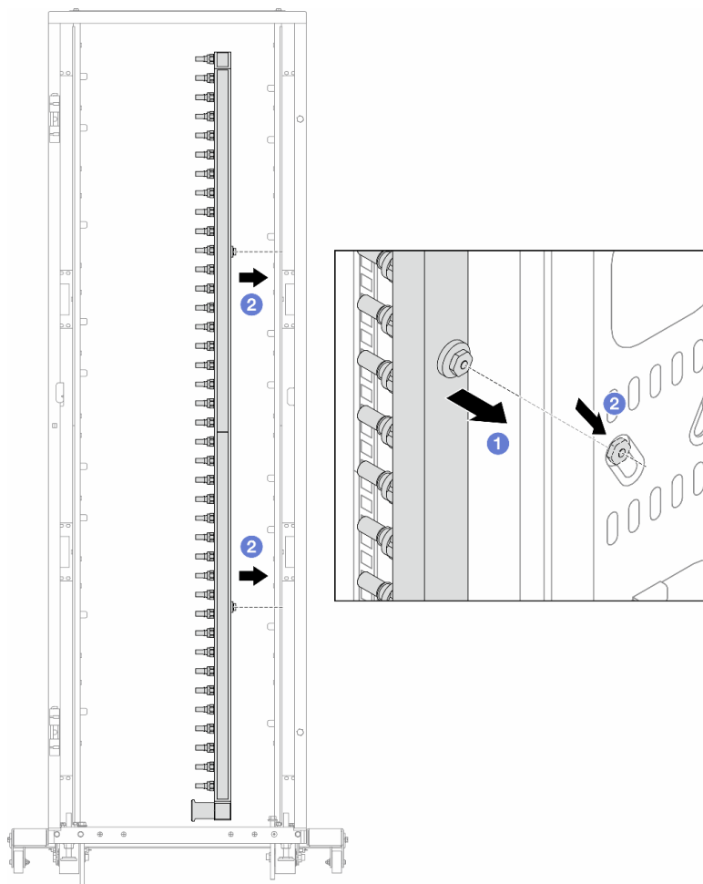
圖例 163. 安裝歧管
