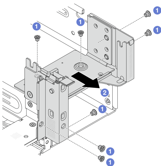
圖例 234. 卸下右側後壁托架
