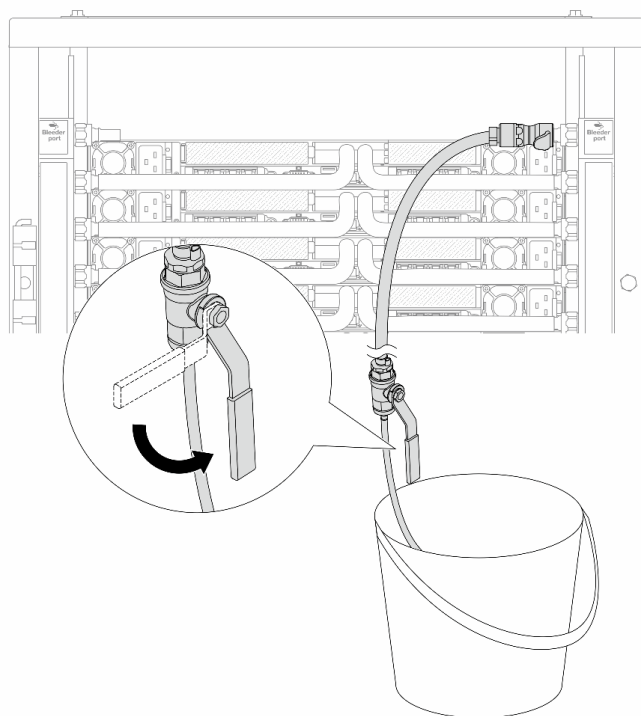
圖例 175. 開啟回流側的洩放閥門
