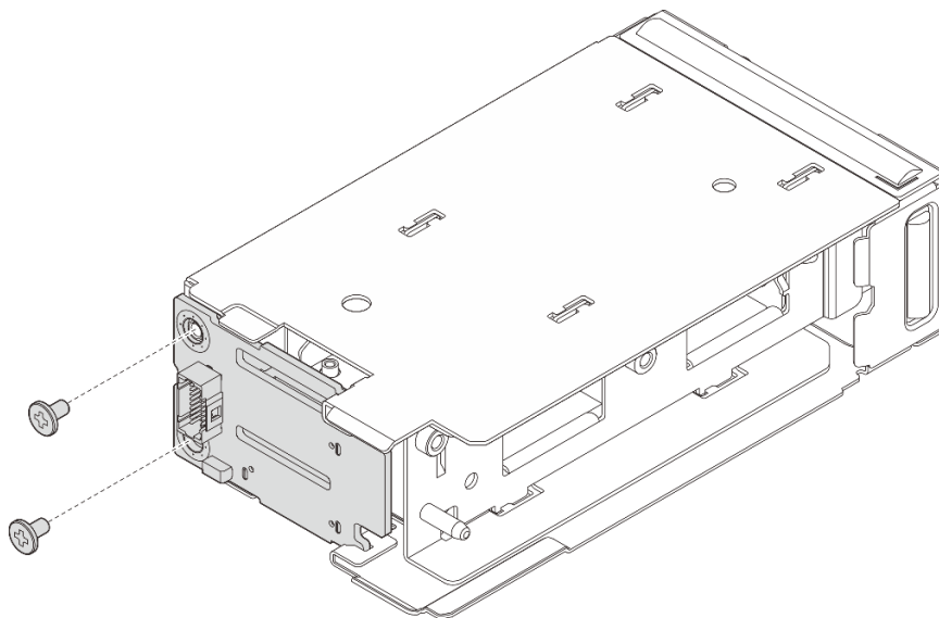
圖例 135. 卸下前方 M.2 開機背板
