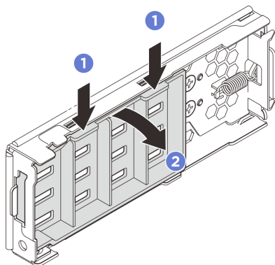
圖例 57. 卸下內板
