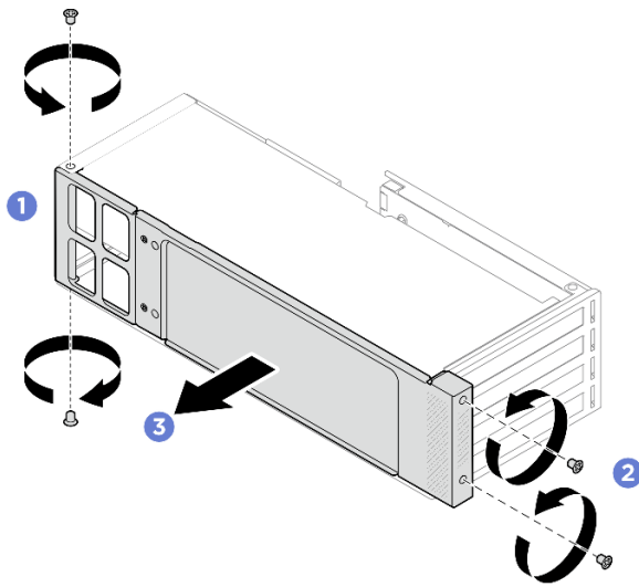
圖例 67. 卸下側面支撐托架
