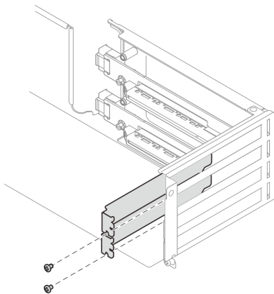
圖例 70. PCIe 插槽填充板
