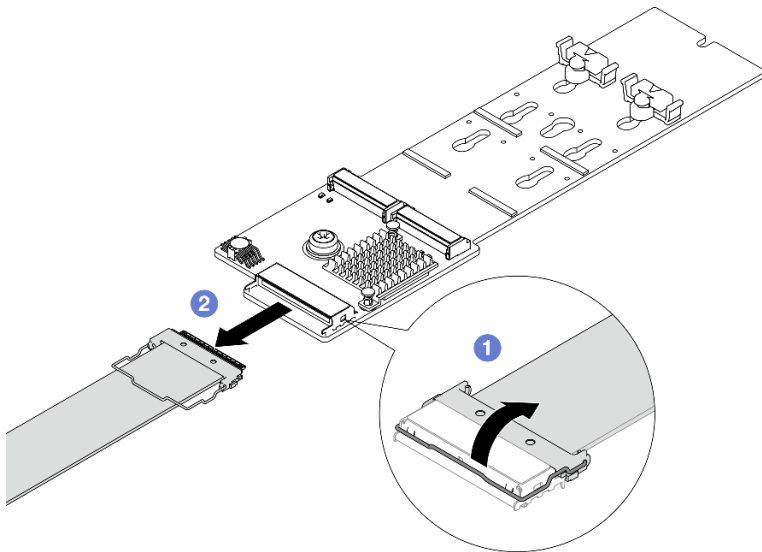
圖例 96. 拔掉 M.2 纜線
