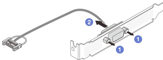
圖例 240. 拆卸序列埠模組
