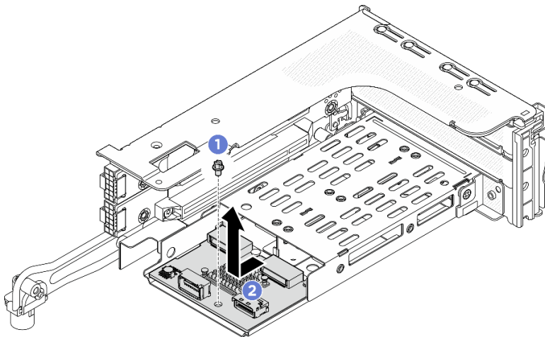
圖例 144. 從 3FH M.2 擴充卡匣中卸下 M.2 背板
