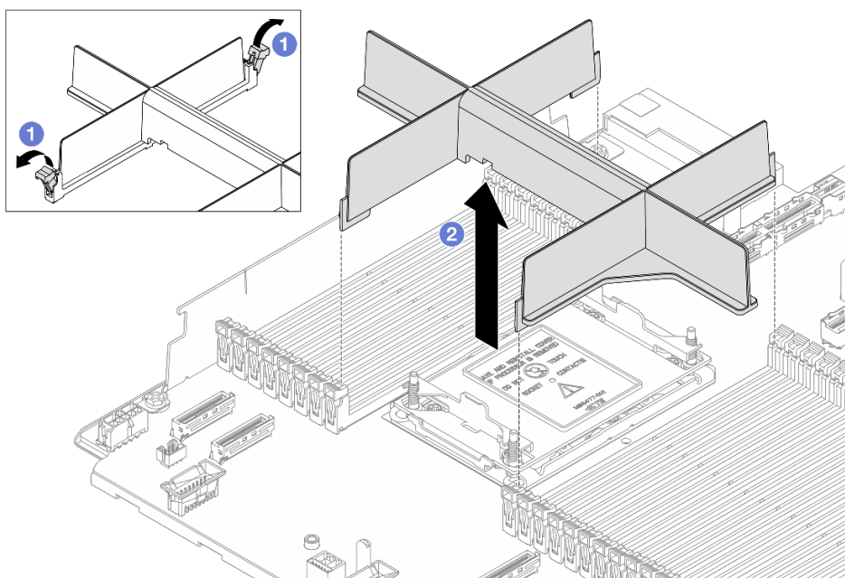
圖例 210. 卸下 PHM 填充板
