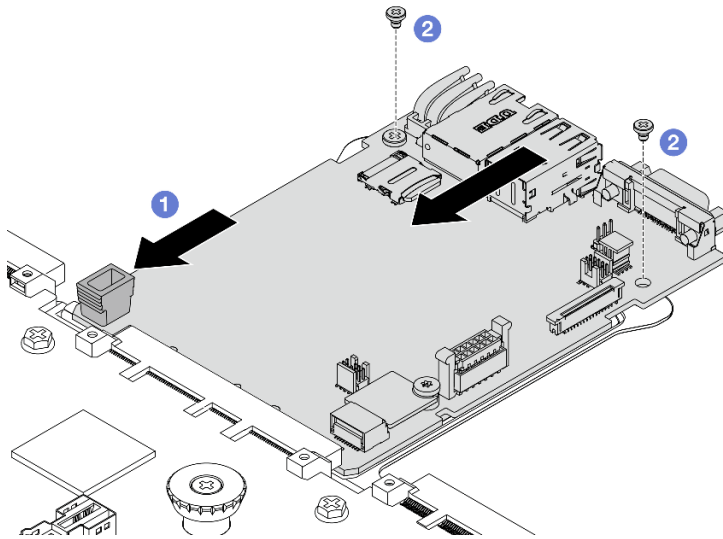
圖例 247. 將系統 I/O 板安裝在處理器板上
