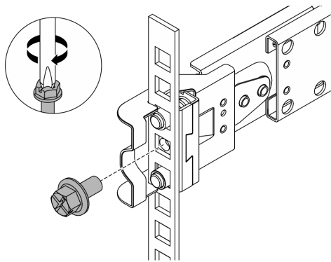
圖例 31. 將伺服器固定到機架背面
