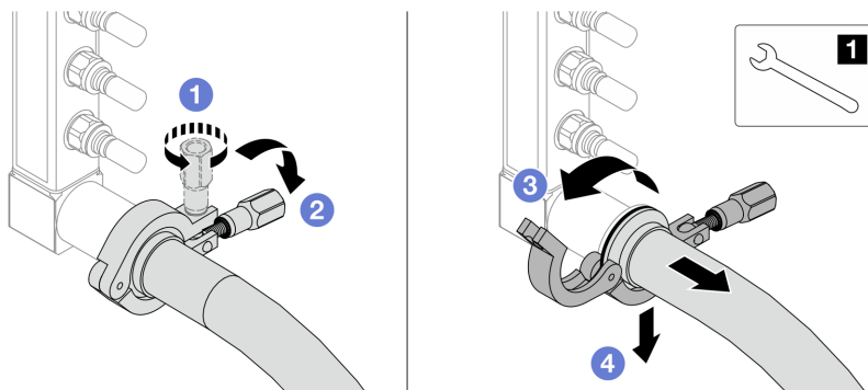
圖例 184. 將歧管與軟管套件分離
