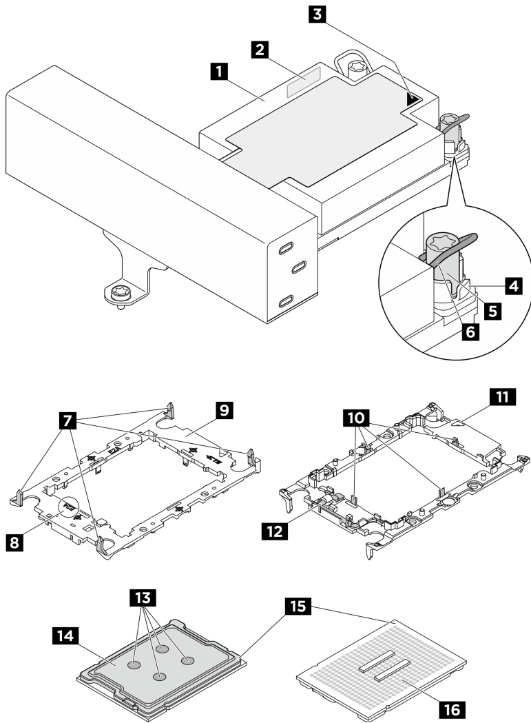
圖例 200. PHM 元件
