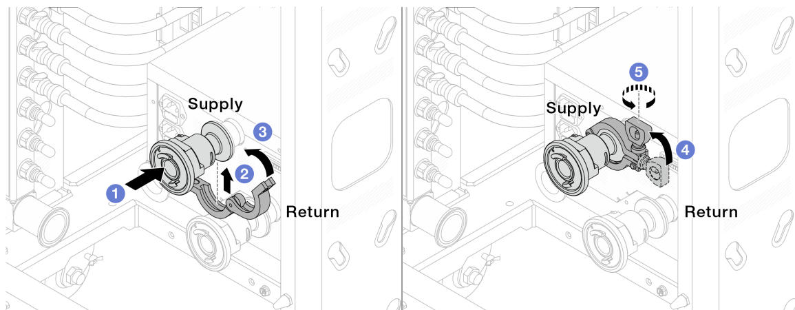
圖例 165. 安裝球閥
