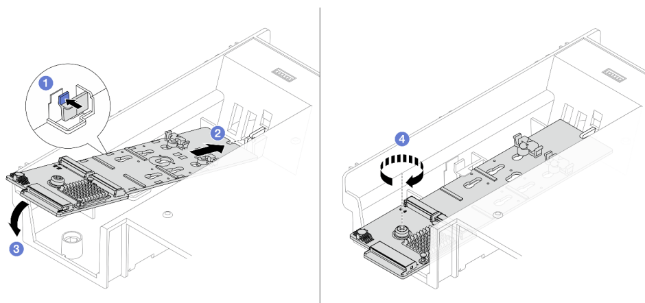
圖例 98. 將 M.2 背板安裝到空氣擋板上
