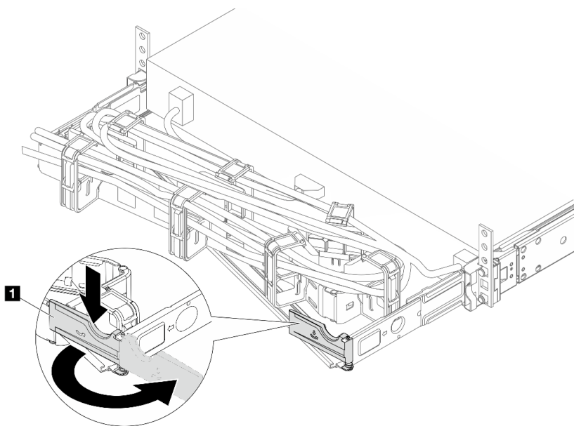
圖例 81. 調整右側
