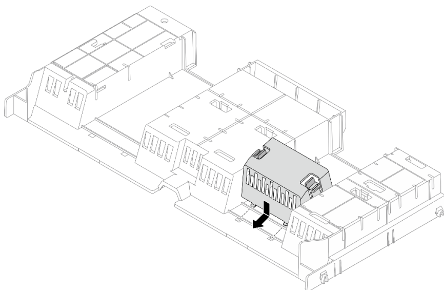
圖例 43. 安裝空氣擋板填充板
