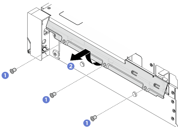
圖例 213. 卸下纜線固定夾
