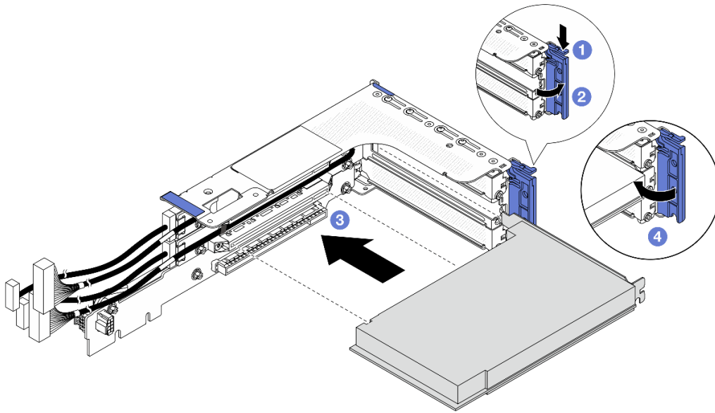
圖例 230. 在 3FH 擴充卡匣上安裝 PCIe 配接卡
