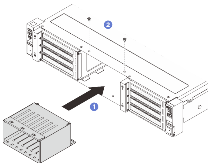
圖例 38. 安裝 2.5 吋框架
