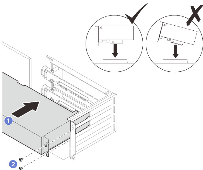
圖例 71. PCIe 配接卡安裝
