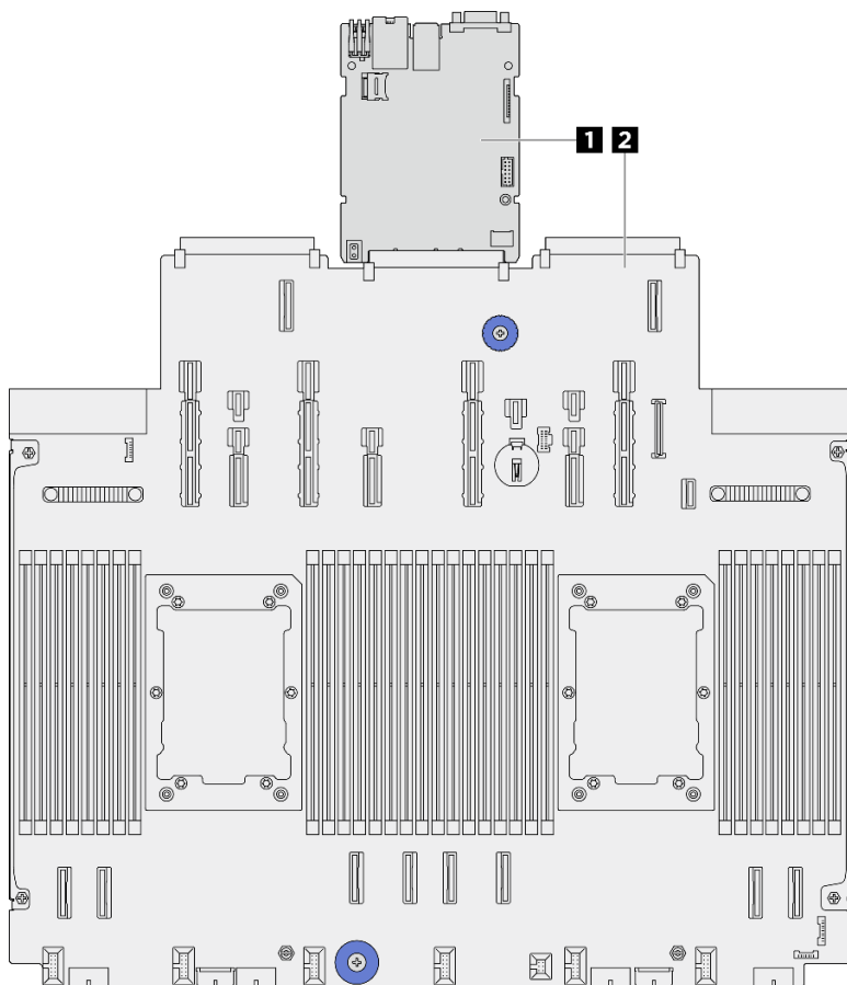
圖例 8. 主機板組件佈置
