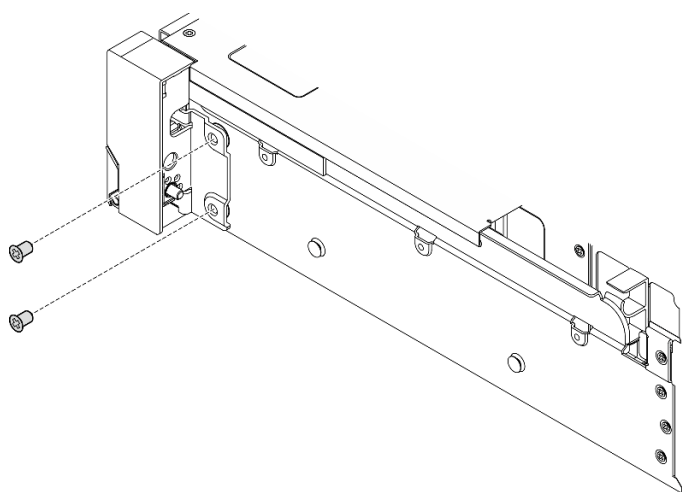
圖例 214. 卸下螺絲
