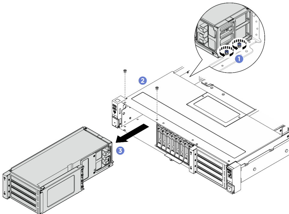
圖例 66. 卸下正面擴充卡組件
