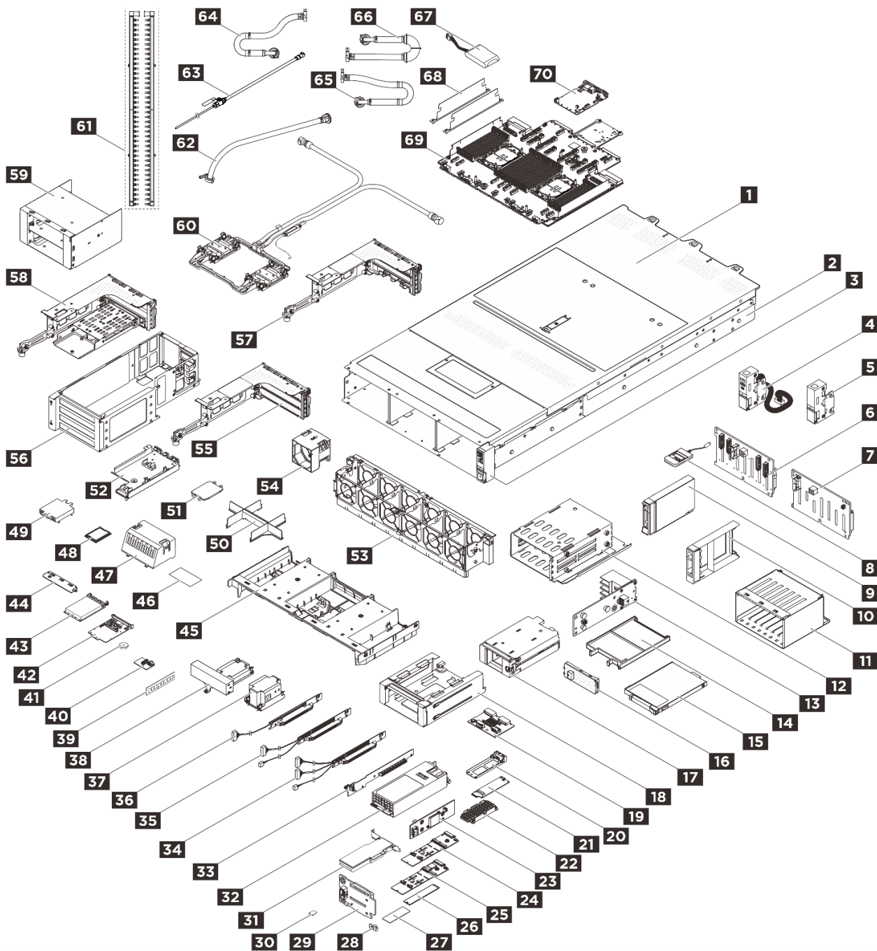
圖例 11. 伺服器元件
