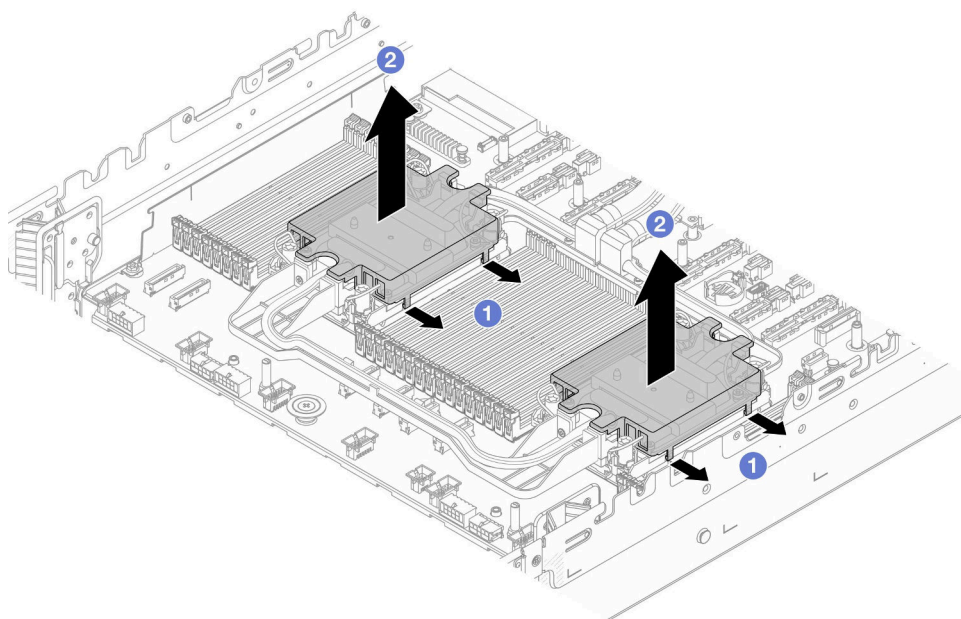
圖例 277. 拆下水冷板蓋
