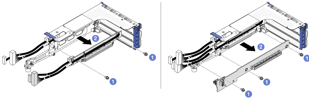
圖例 228. 從擴充卡匣卸下擴充卡
