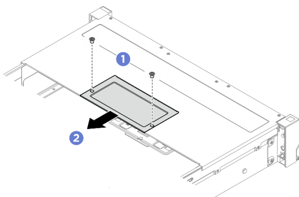
圖例 59. 卸下蓋板
