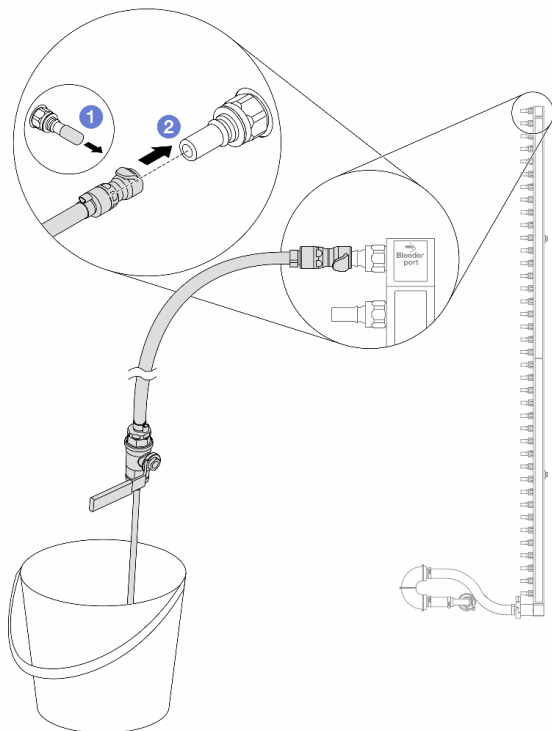
圖例 160. 在回流側安裝洩放套件
