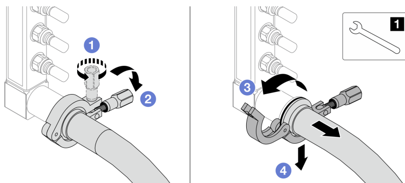
圖例 162. 將歧管與連接套組分開
