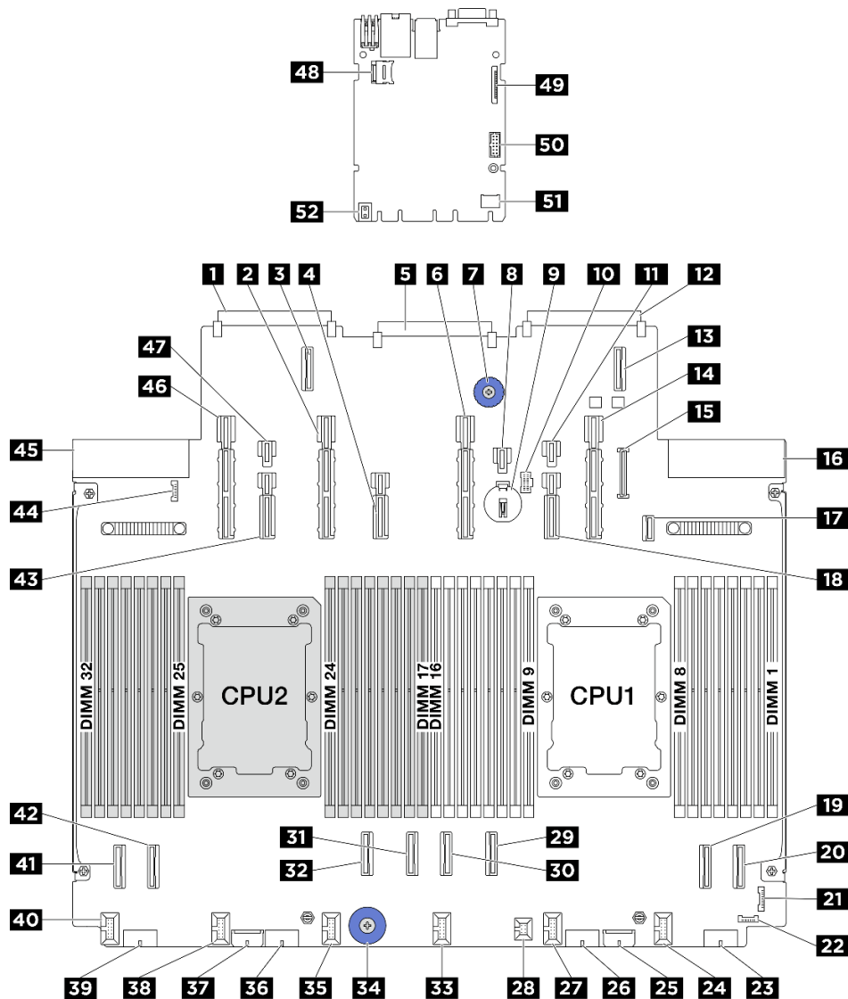
圖例 9. 主機板組件接頭
