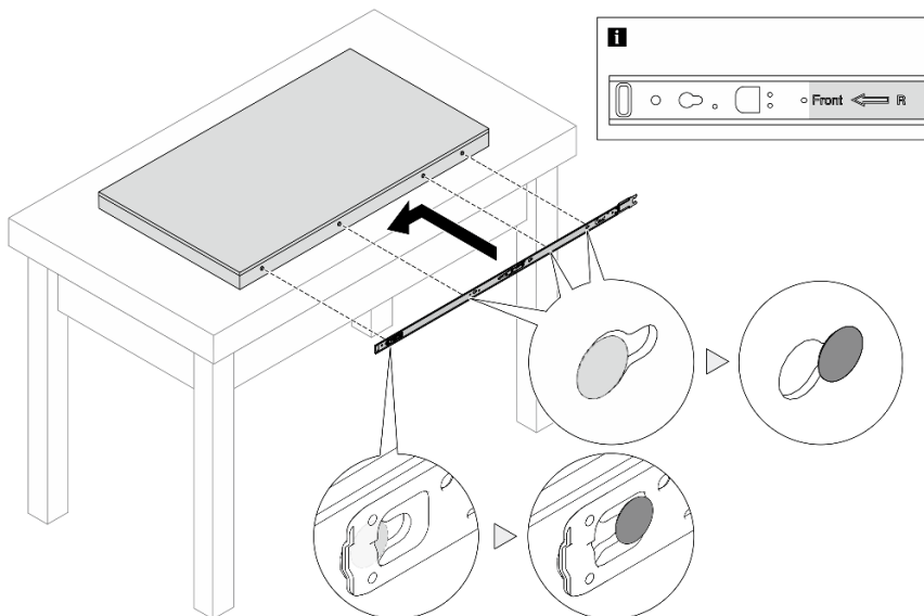
圖例 26. 安裝內滑軌
