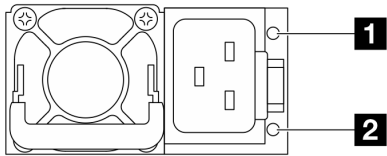
圖例 271. CRPS Premium 電源供應器上的 LED
