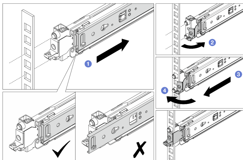
圖例 20. 安裝前方安裝插腳
