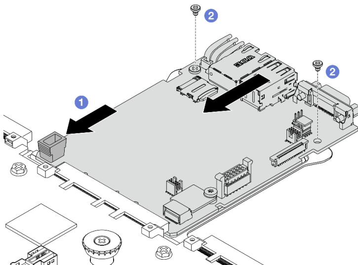
圖例 251. 將系統 I/O 板安裝在處理器板上
