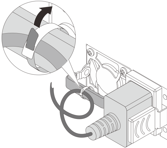
圖例 88. 佈線和固定電源線
