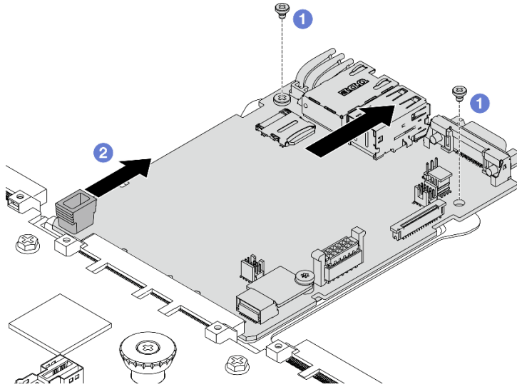
圖例 250. 將系統 I/O 板與處理器板分開
