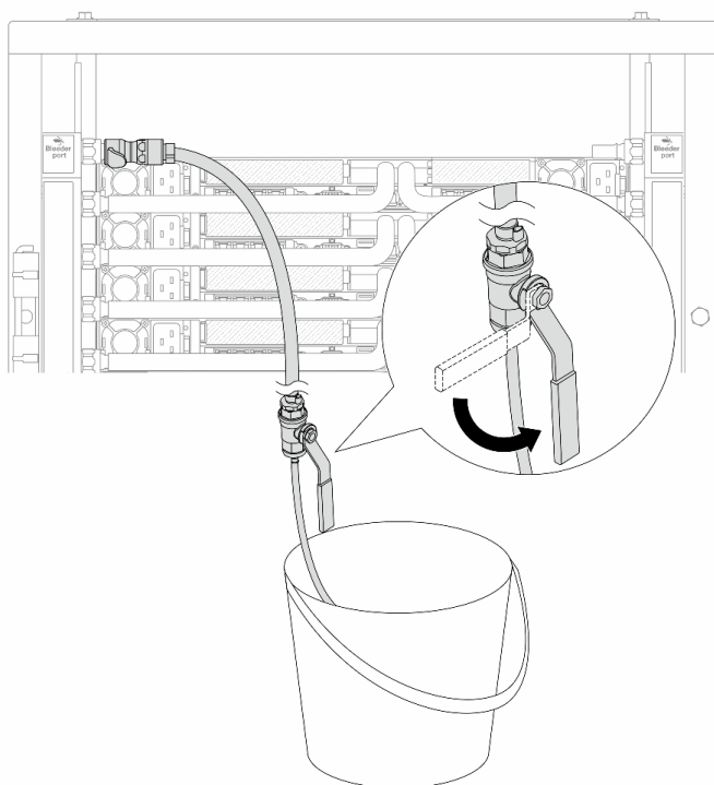
圖例 173. 開啟供應側的洩放閥門
