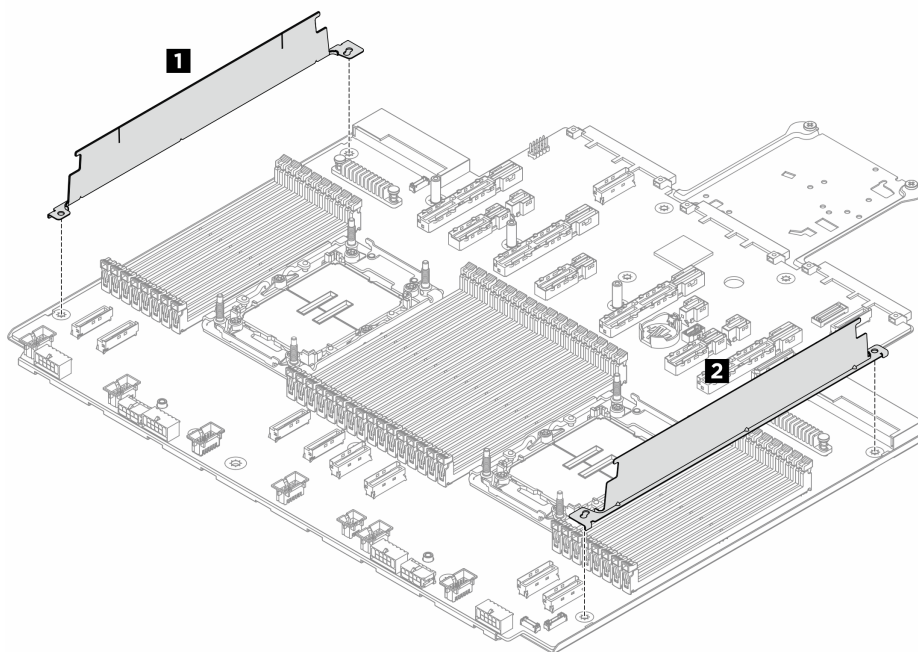
圖例 279. 卸下纜線壁
