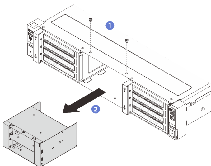
圖例 62. 卸下 E3.S 框架
