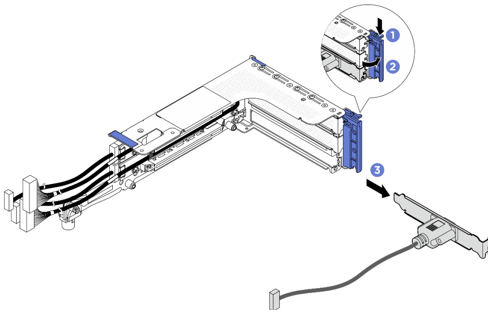
圖例 239. 卸下序列埠模組
