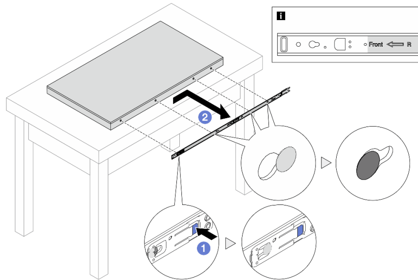
圖例 24. 卸下內滑軌
