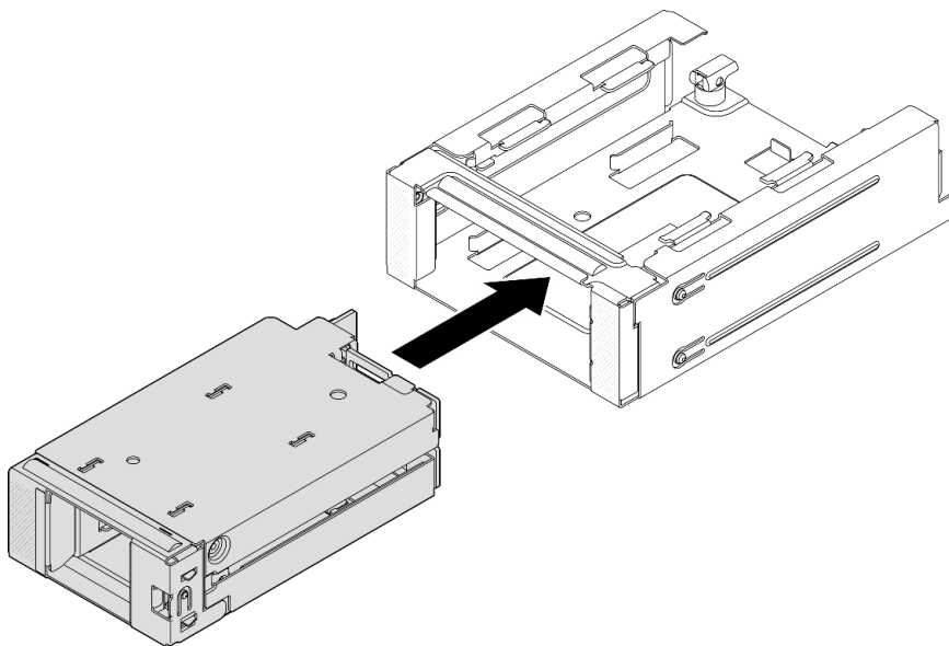
圖例 141. 將前方 M.2 框架安裝至機架中
