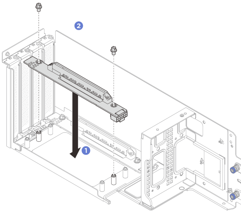
圖例 77. 擴充卡安裝
