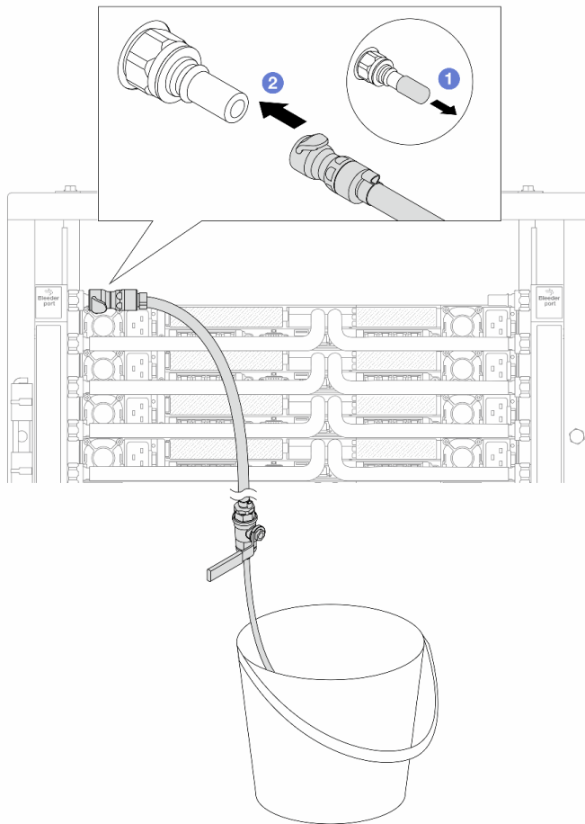
圖例 171. 安裝供應側的洩放套件
