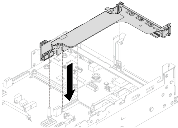
Abbildung 237. Installieren der Adapterkartenbaugruppe
