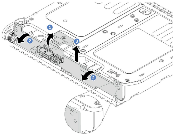
Abbildung 207. Entfernen der hinteren Rückwandplatine für 2 x 3,5-Zoll-Laufwerke
