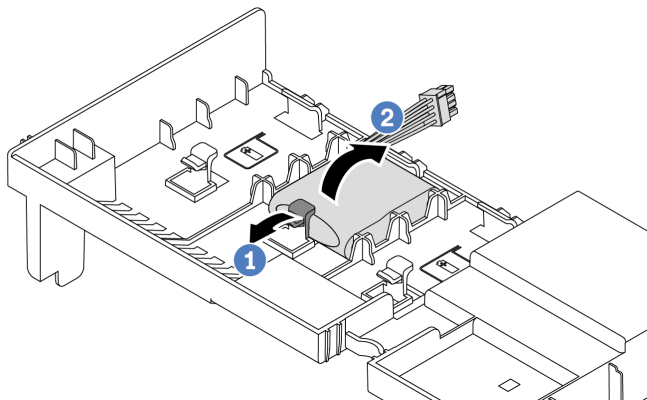
Abbildung 172. Entfernen des RAID-Flash-Stromversorgungsmoduls von der Luftführung
