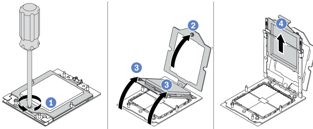
Abbildung 148. Entfernen eines Prozessors
