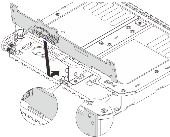
Abbildung 208. Installieren der hinteren Rückwandplatte für 2 x 3,5-Zoll-Laufwerke
