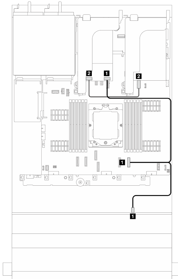
Abbildung 260. Kabelführung der Rückwandplatine für 7-mm-Laufwerke in Konfiguration mit 12 x 3,5-Zoll-SAS/SATA-Rückwandplatine
