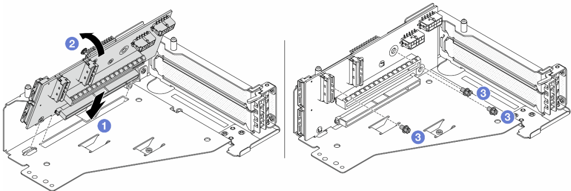
Abbildung 26. Installieren der Adapterkarte
