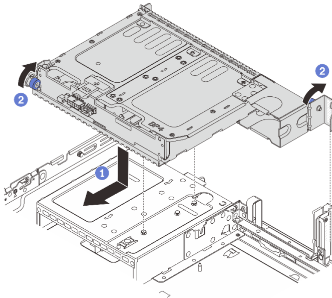
Abbildung 209. Hintere 2 x 3,5-Zoll-Laufwerkhalterung installieren
