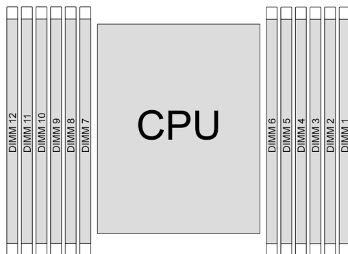
Abbildung 1. Layout für Speichermodule und Prozessoren
