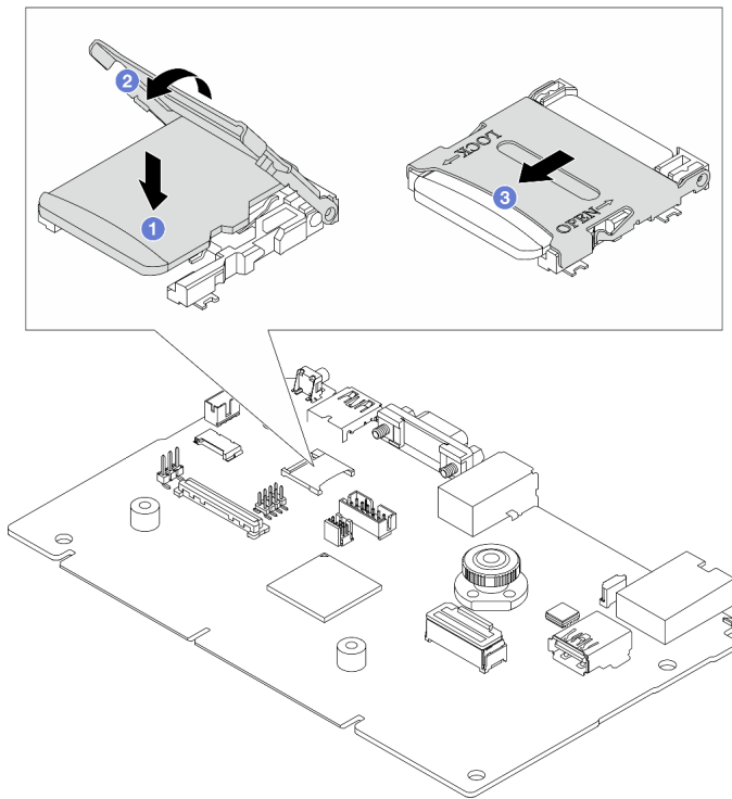
Abbildung 108. Installieren der microSD-Karte
