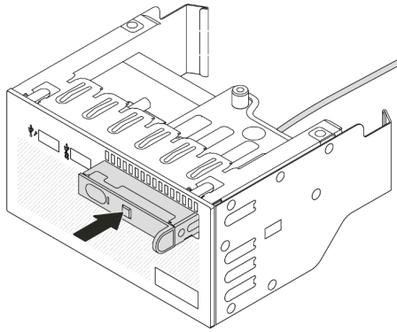
Abbildung 65. Installieren der integrierten Diagnoseanzeige
