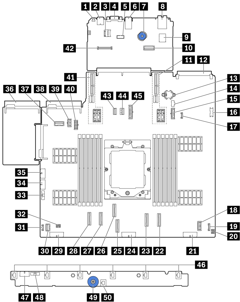
Abbildung 389. Anschlüsse auf der Systemplatinenbaugruppe
