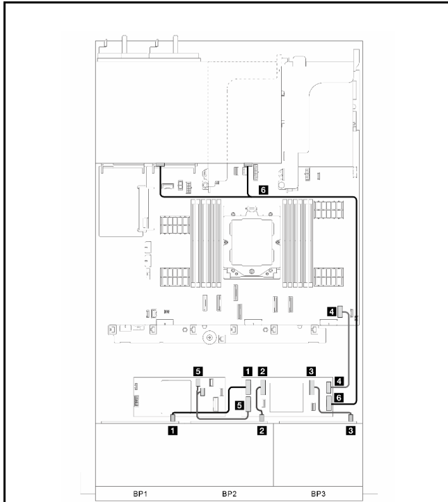
Abbildung 335. Signalkabelführung Teil 1
