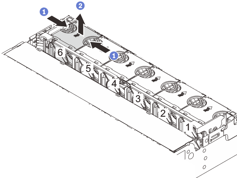
Abbildung 227. Systemlüfter entfernen
