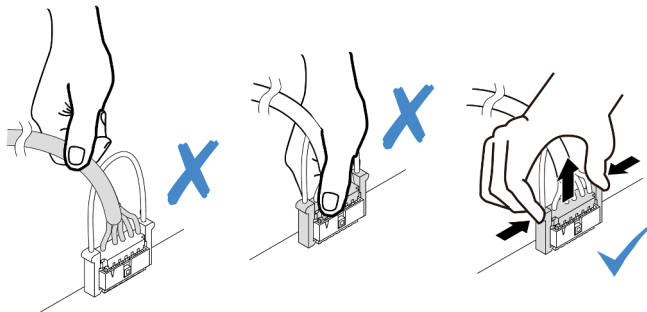
Abbildung 231. Trennen des Kabels von der System-E/A-Karte
