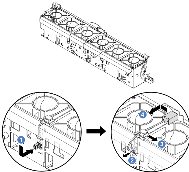
Abbildung 87. Entfernen des Schalters gegen unbefugten Zugriff
