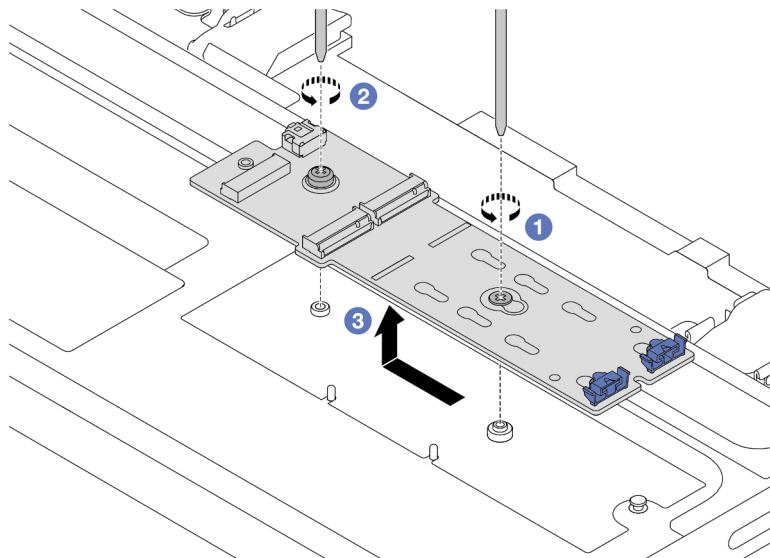
Abbildung 97. Entfernen der M.2-Rückwandplatte aus der mittleren Laufwerkhalterung
