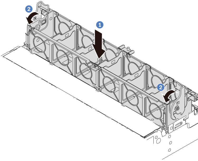
Abbildung 230. Systemlüfterrahmen installieren
