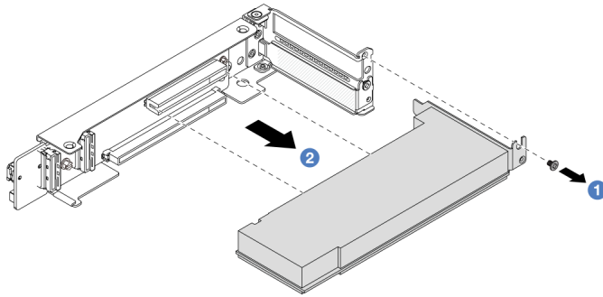
Abbildung 121. Entfernen eines PCIe-Adapters aus der 4LP-3/4-Adapterkartenbaugruppe
