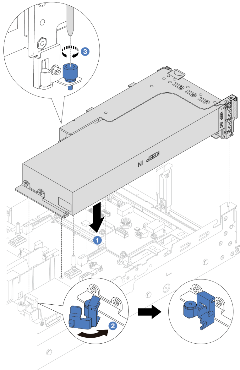
Abbildung 75. Installieren der Adapterkartenbaugruppe 1 mit GPU-Adapter
