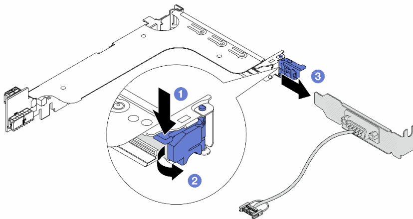
Abbildung 233. Entfernen des seriellen Anschlussmoduls
