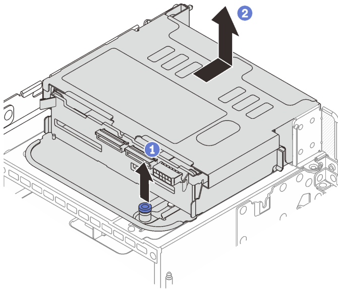
Abbildung 198. Entfernen der hinteren 4 x 2,5-Zoll-Laufwerkhalterung
