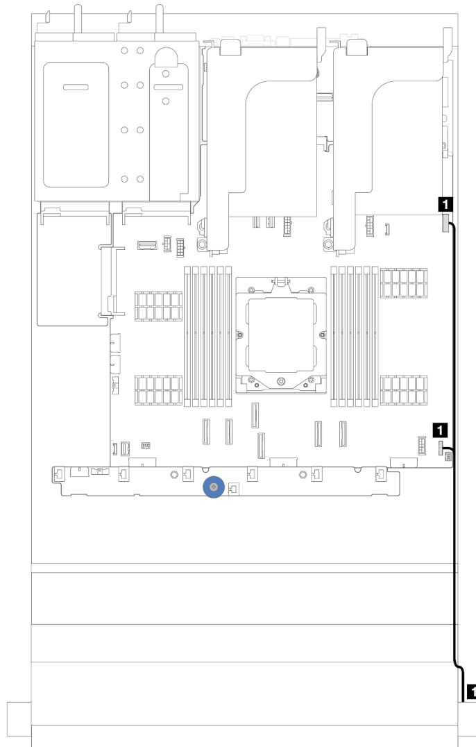
Abbildung 261. Kabelführung für das E/A-Modul an der rechten Rack-Verriegelung
