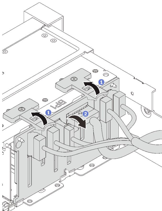
Abbildung 52. Entfernen der Rückwandplatte für 2,5-Zoll-Laufwerke
