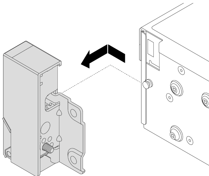
Abbildung 156. Entfernen der Rack-Verriegelung
