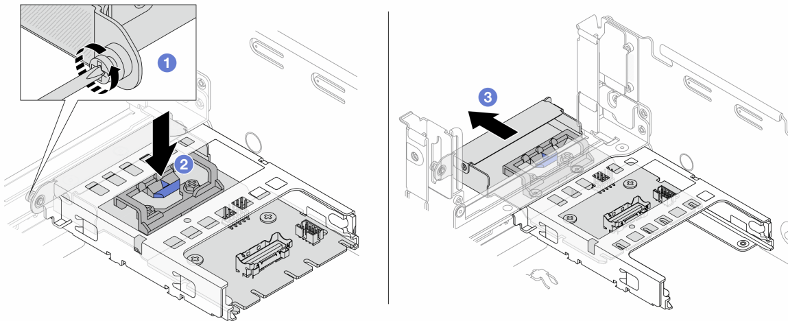
Abbildung 40. Entfernen der hinteren OCP-Interposerkarte
