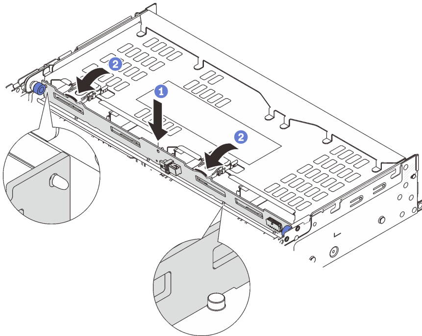
Abbildung 212. Installieren der hinteren Rückwandplatine für 4 x 3,5-Zoll-Laufwerke
