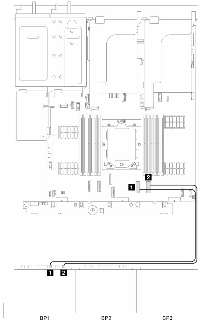
Abbildung 297. Integrierte Anschlüsse (unterstützt Adapterkarte 3)
