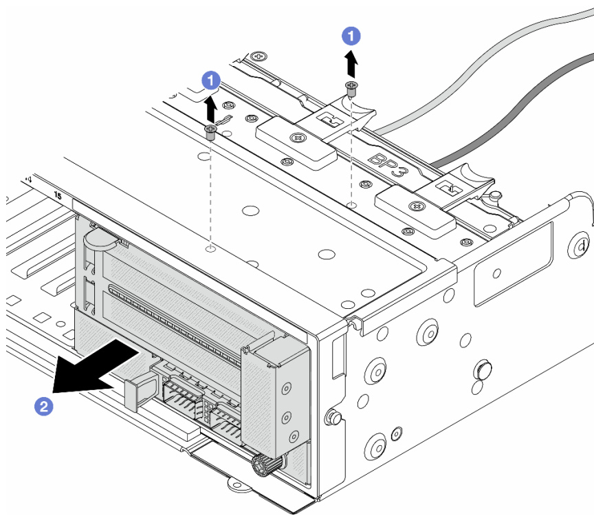
Abbildung 42. Entfernen der vorderen Adapterbaugruppe
