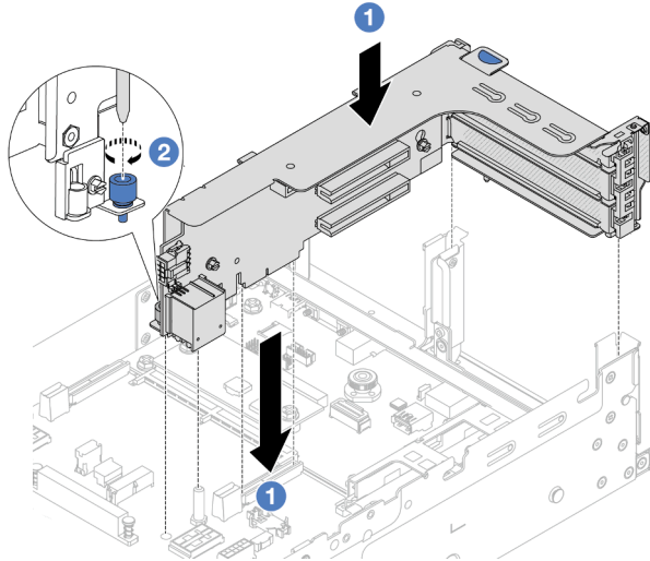
Abbildung 131. Installieren der Adapterkartenbaugruppe 1
