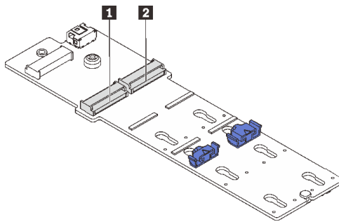
Abbildung 91. M.2-Laufwerksteckplatz
