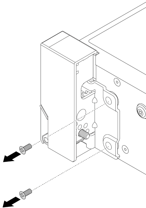
Abbildung 155. Entfernen der Schrauben
