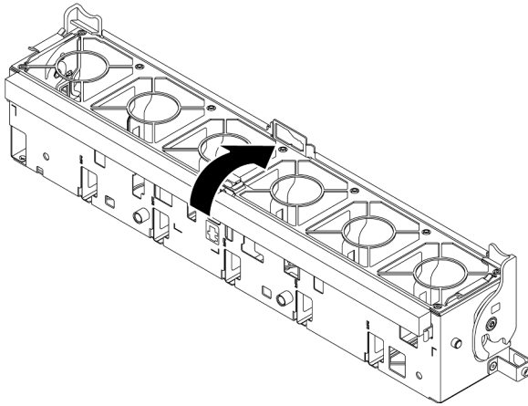
Abbildung 86. Drehen des Lüfterrahmens
