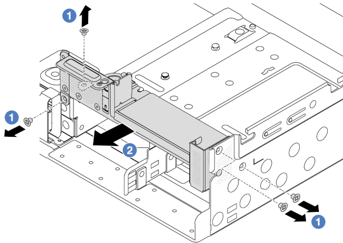
Abbildung 182. Entfernen der Rückwandhalterung C1 (rechts)
