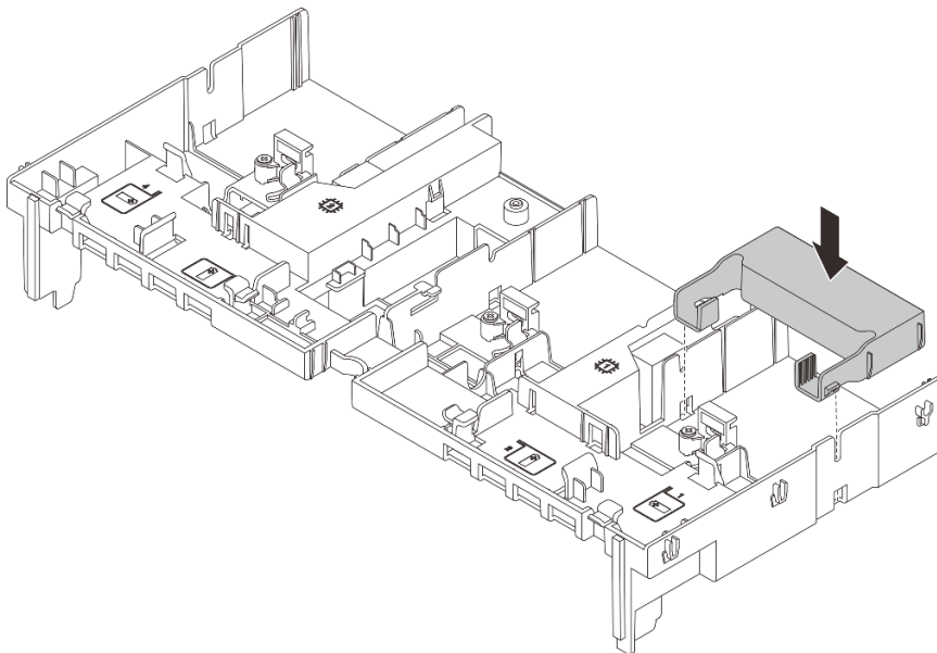
Abbildung 74. Installieren einer zusätzlichen Luftführung
