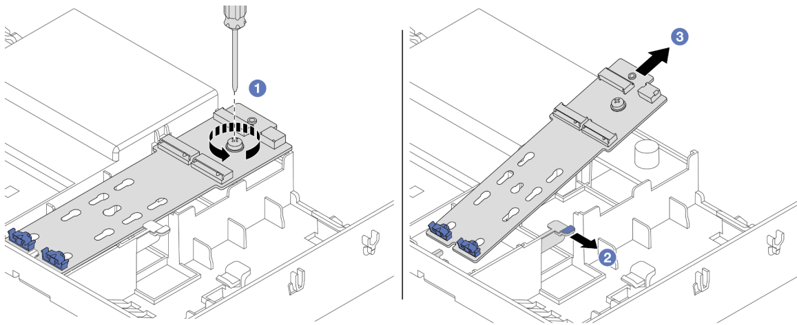
Abbildung 96. Entfernen der M.2-Rückwandplatte von der Luftführung
