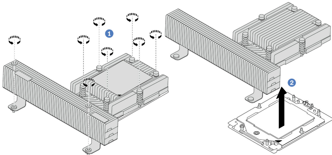
Abbildung 147. Entfernen eines Hochleistungskühlkörpers
