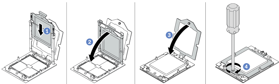
Abbildung 149. Installieren eines Prozessors
