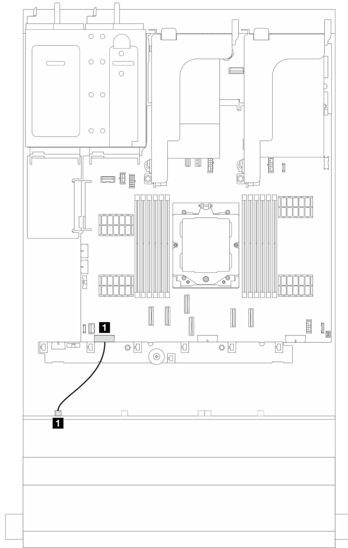
Abbildung 359. Netzkabelführung für die vordere Expander-Rückwandplatine für 12 x 3,5-Zoll-SAS/SATA-Laufwerke
