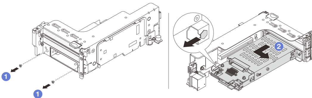
Abbildung 188. Entfernen Sie die 7-mm-Laufwerkhalterung aus der Adapterkartenbaugruppe.
