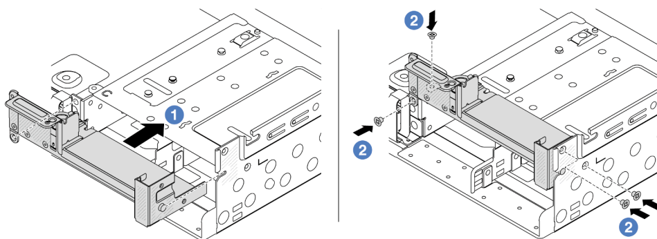
Abbildung 185. Installieren der Rückwandhalterung C1 (rechts)
