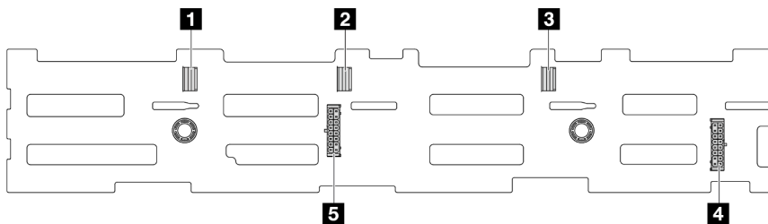
Abbildung 245. Anschlüsse an der 12 x 3,5-Zoll-SAS/SATA-Rückwandplatine
