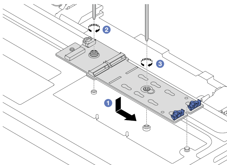
Abbildung 99. Installieren der M.2-Rückwandplatine an der mittleren Laufwerkhalterung
