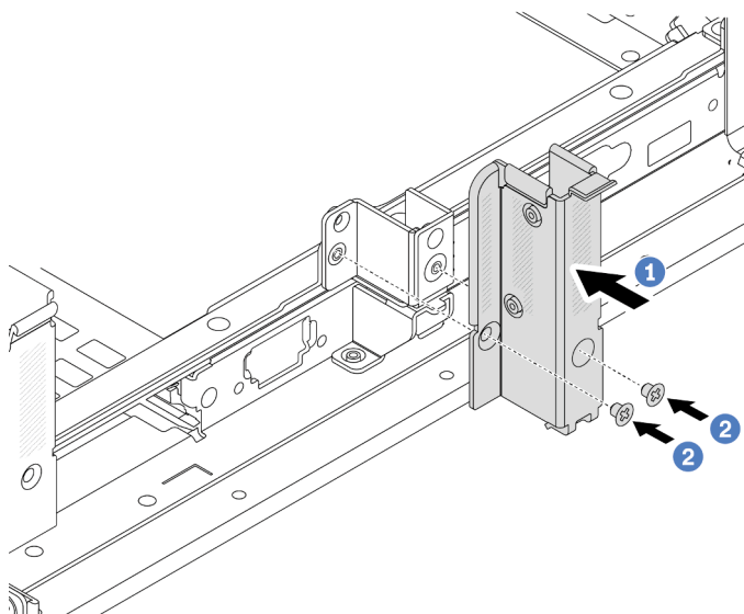
Abbildung 184. Installieren der Rückwandhalterung B1 (Mitte)
