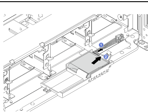
Abbildung 165. Entfernen Sie das RAID-Flash-Stromversorgungsmodul von der Superkondensator-Halterung.
