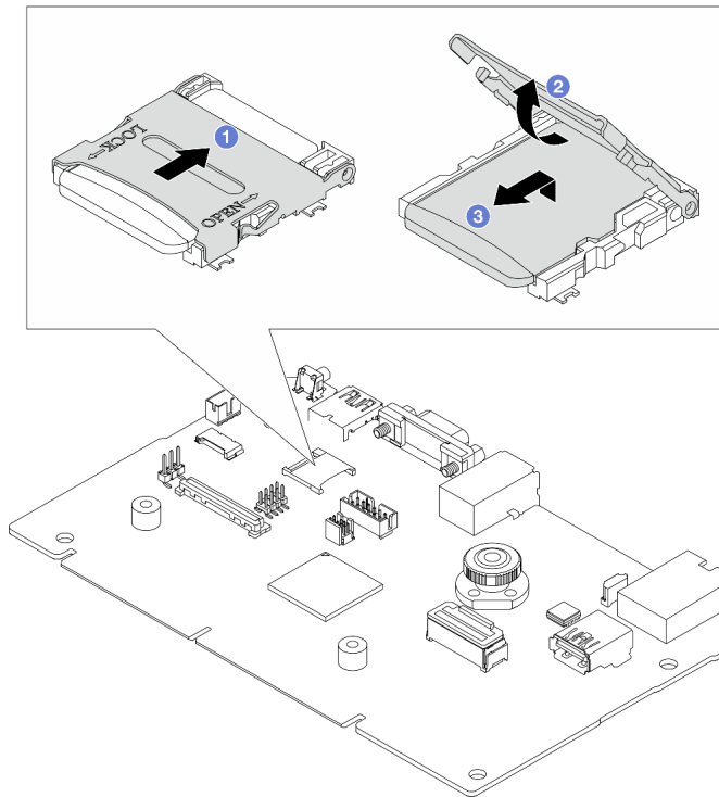
Abbildung 107. Entfernen der microSD-Karte
