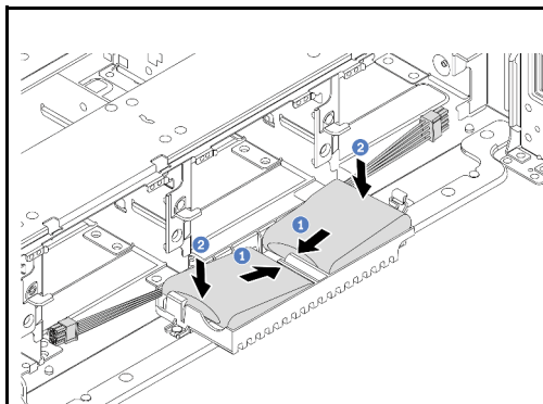
Abbildung 170. Installieren Sie das RAID-Flash-Stromversorgungsmodul auf der Superkondensator-Halterung.
