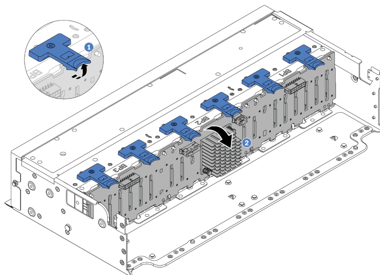
Abbildung 53. Entfernen der Rückwandplatte für Laufwerke mit 24 Positionen
