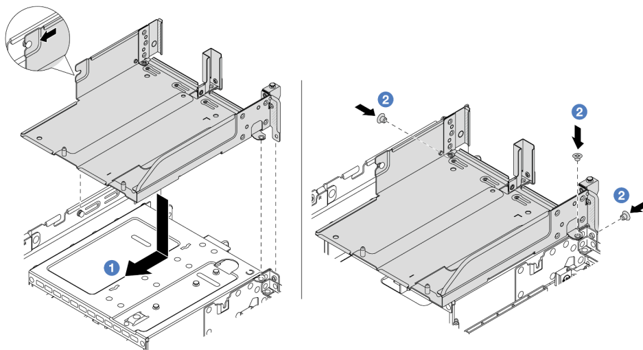
Abbildung 133. Installieren Sie den Adaptereinbaurahmen.
