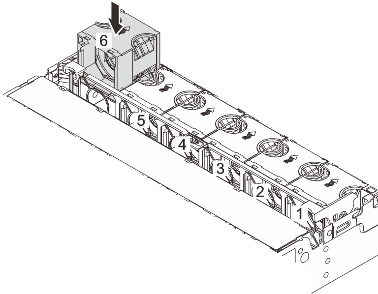
Abbildung 228. Installieren des Systemlüfters
