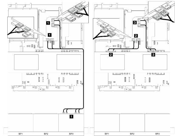
Abbildung 352. Signalkabelführung Teil 2
