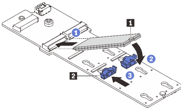
Abbildung 92. M.2-Laufwerk installieren
