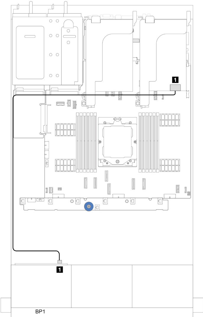
Abbildung 298. SAS/SATA-Kabelführung zum 8i/16i RAID/HBA-Adapter
