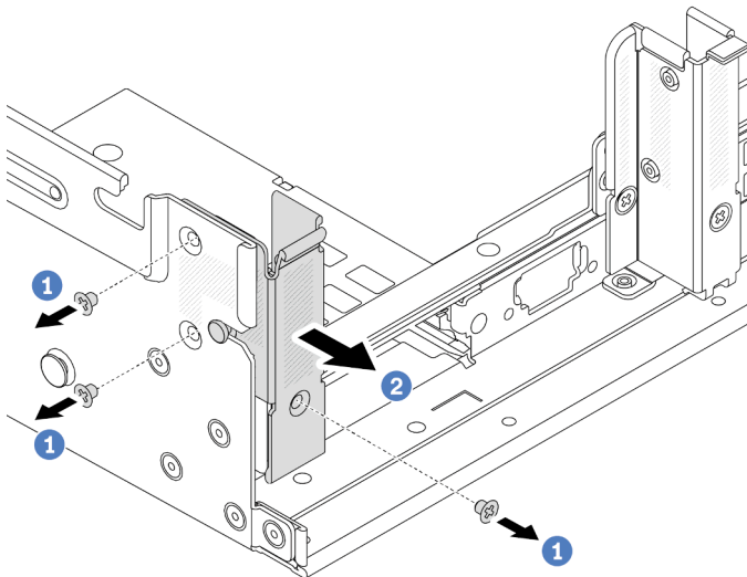
Abbildung 180. Entfernen der Rückwandhalterung A1 (links)
