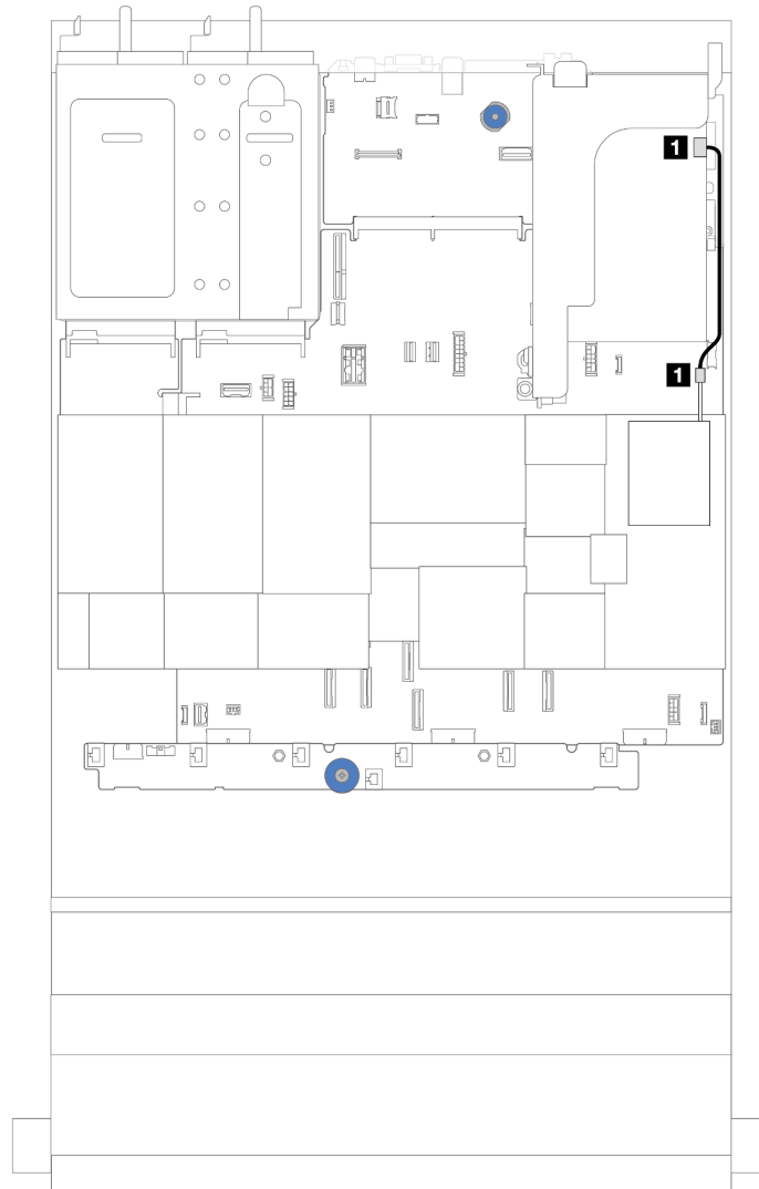
Abbildung 276. Kabelführung für RAID-Flash-Stromversorgungsmodul
