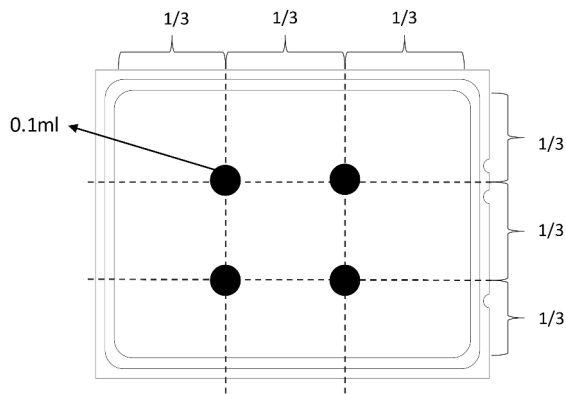
Abbildung 150. Wärmeleitpaste auftragen
