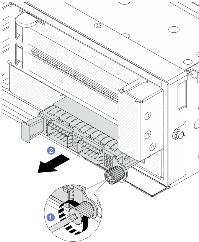
Abbildung 30. Entfernen des vorderen OCP-Moduls
