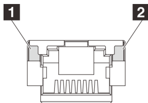
Abbildung 392. Anzeigen am XCC-Systemmanagement-Anschluss
