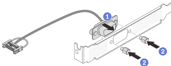
Abbildung 235. Montieren des seriellen Anschlussmoduls
