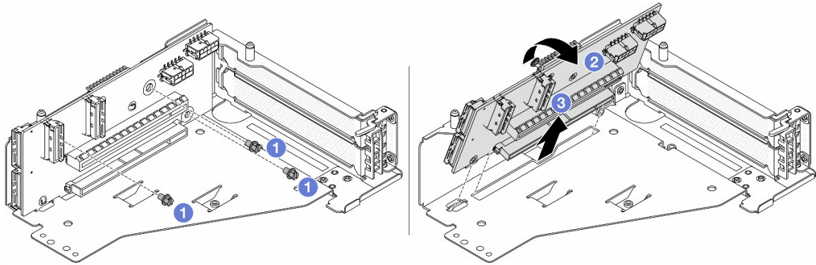
Abbildung 45. Entfernen der Adapterkarte aus Adapterrahmen 5
