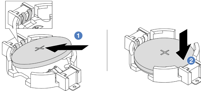
Abbildung 17. Installieren der CMOS-Batterie
