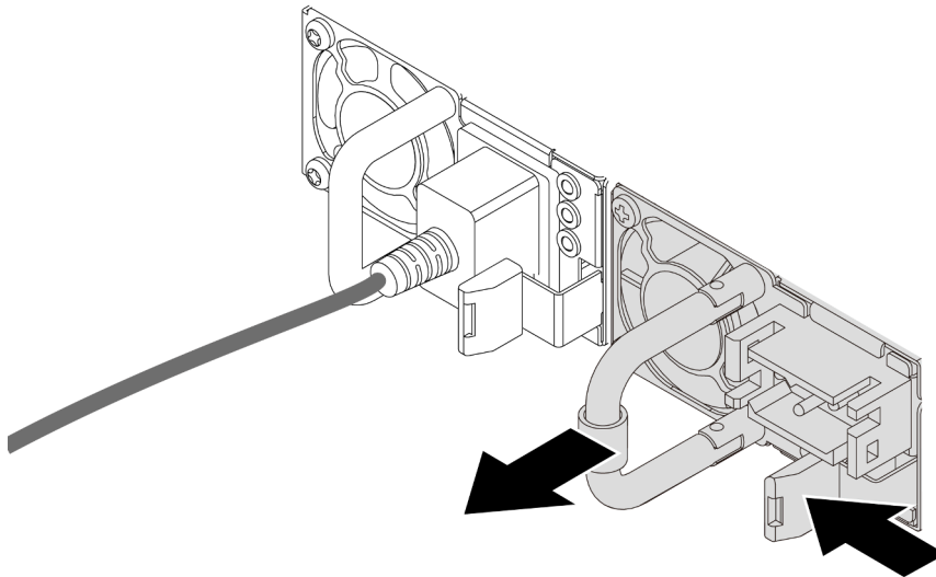
Abbildung 142. Entfernen der Netzteilereinheit
