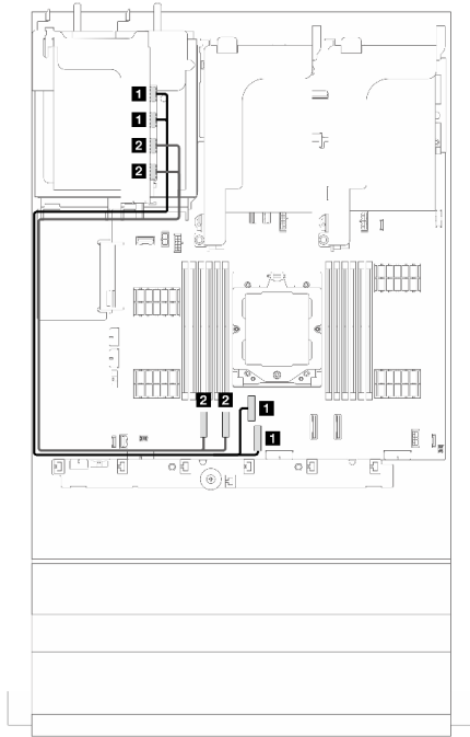
Abbildung 278. Signalkabelführung für Adapterkarte 3 (x16/x16 Gen 5)
