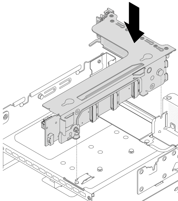
Abbildung 132. Installieren der Adapterkartenbaugruppe 3
