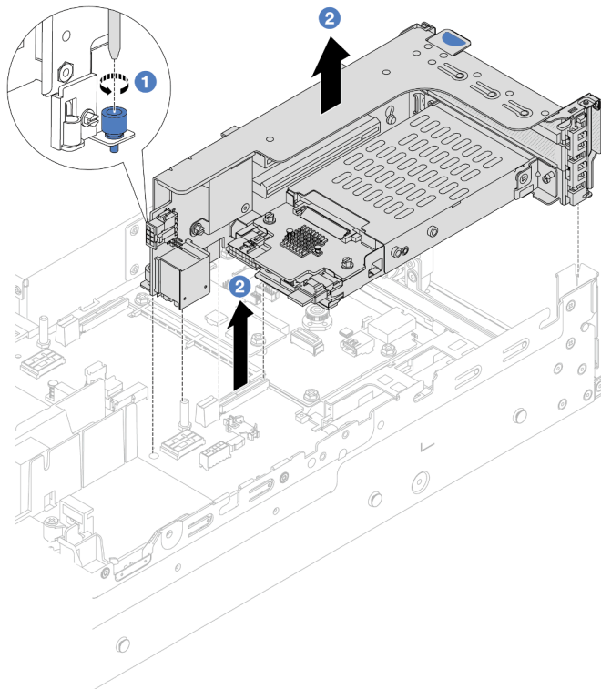
Abbildung 186. Entfernen des 2FH+7 mm SSD-Adapterrahmens
