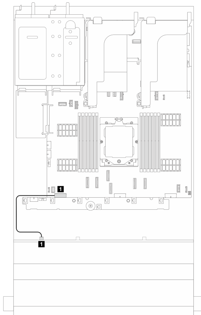
Abbildung 357. Netzkabelführung für die 8 x 3,5-Zoll-SAS/SATA-Rückwandplatte
