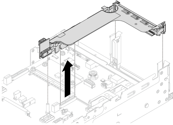
Abbildung 232. Entfernen der Adapterkartenhalterung
