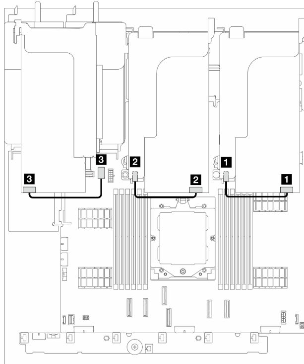
Abbildung 263. Kabelführung für GPU-Adapter
