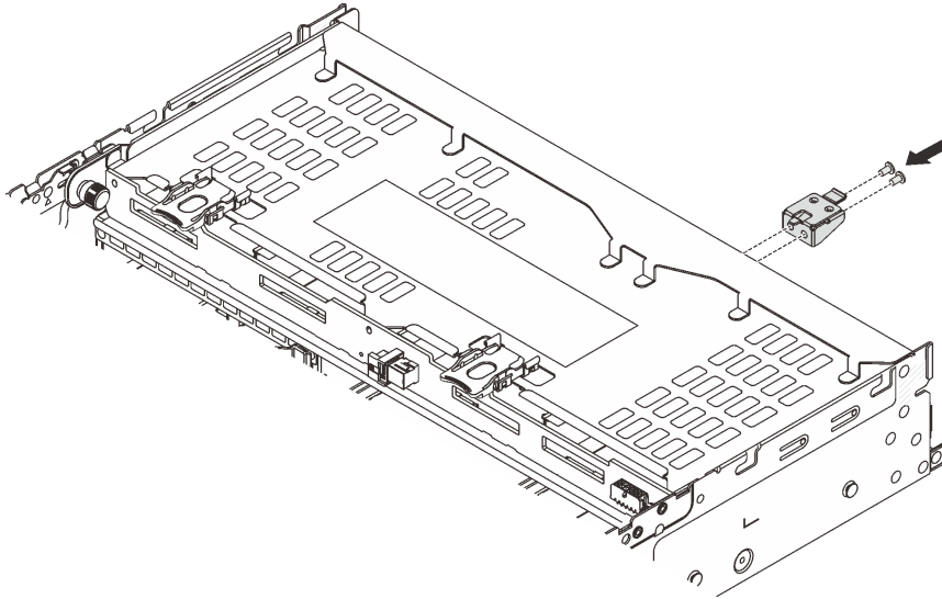
Abbildung 214. Installieren des Stützwinkels der oberen Abdeckung
