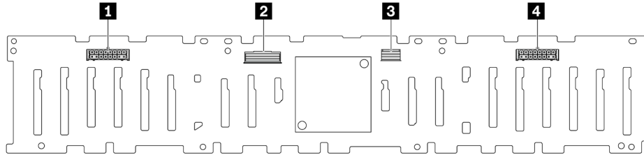
Abbildung 243. Anschlüsse an der 24 x 2,5-Zoll-SAS/SATA-Expander-Rückwandplatine
