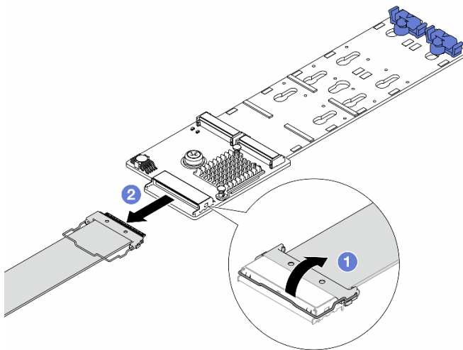
Abbildung 95. Abziehen der M.2-Kabel von ThinkSystem M.2 RAID B540i-2i SATA/NVMe Enablement Kit
