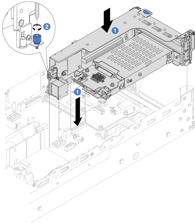
Abbildung 196. Installieren des 2FH+7mm SSD-Adapterrahmens
