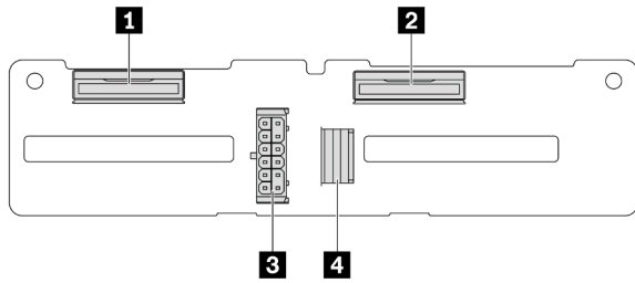
Abbildung 253. Anschlüsse an der 4 x 2,5-Zoll-AnyBay-Rückwandplatine
