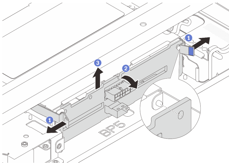
Abbildung 110. Entfernen der mittleren Rückwandplatine für 2,5-Zoll-Laufwerke
