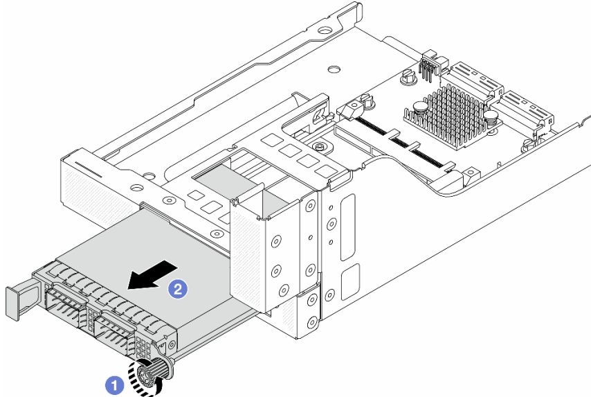
Abbildung 34. Herausnehmen des OCP-Moduls
