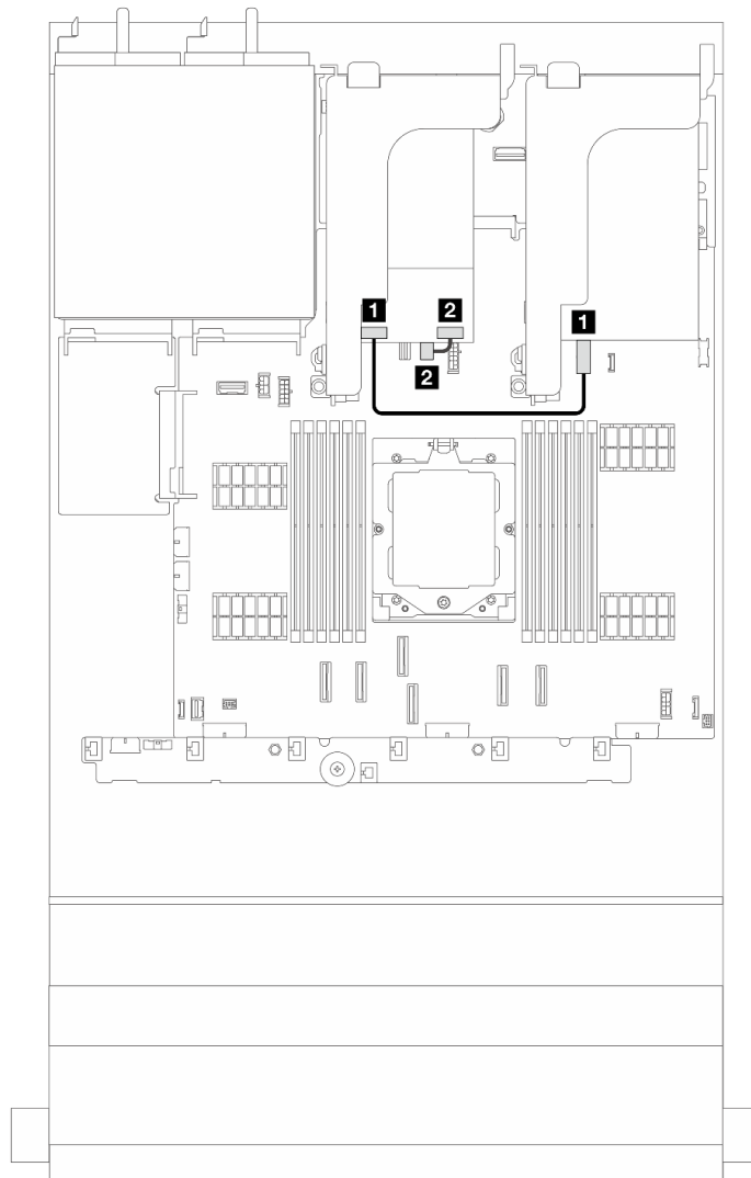
Abbildung 259. Kabelführung für Rückwandplatinen für 7-mm-Laufwerke
