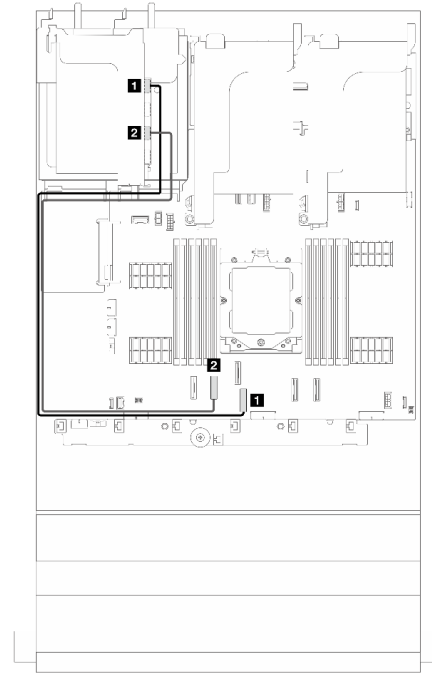
Abbildung 279. Signalkabelführung für Adapterkarte 3 (x8/x8 Gen 5)
