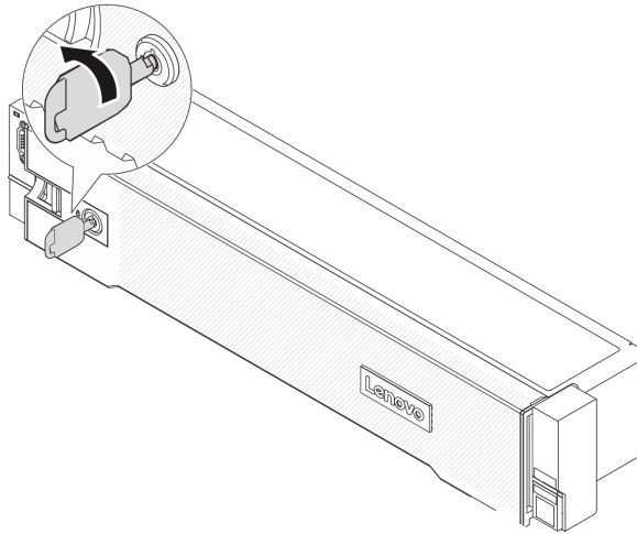
Abbildung 219. Sicherheitsfrontblende verriegeln
