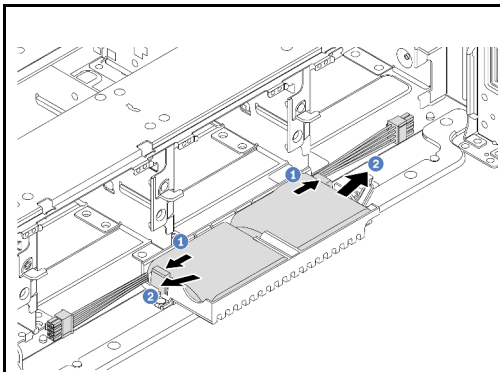
Abbildung 164. Entfernen Sie das RAID-Flash-Stromversorgungsmodul von der Superkondensator-Halterung.
