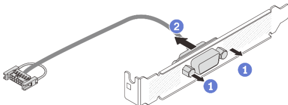
Abbildung 234. Zerlegen des seriellen Anschlussmoduls
