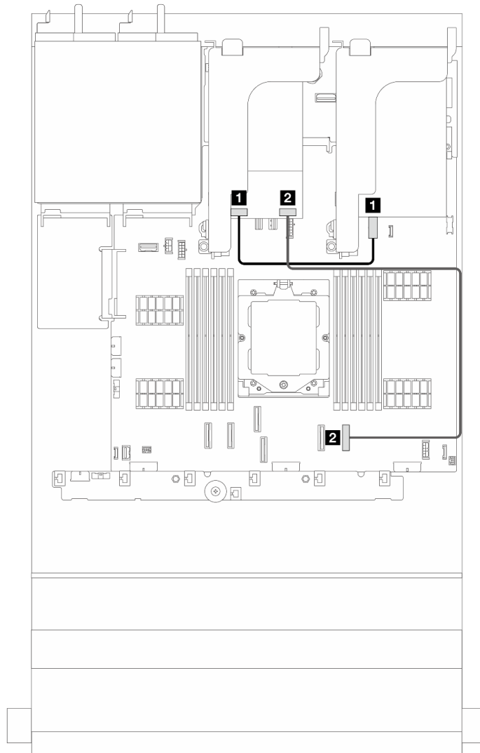
Abbildung 255. SATA-Kabelführung für Rückwandplatten für 7-mm-Laufwerke
