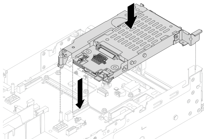
Abbildung 197. Installieren des 7mm-SSD-Adapterrahmens
