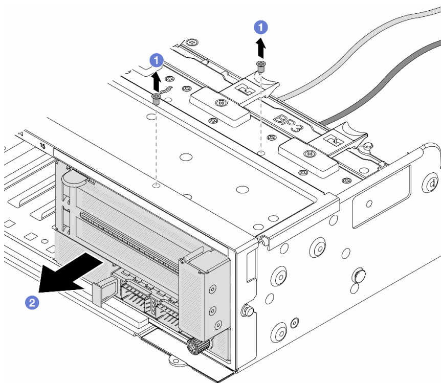
Abbildung 32. Entfernen der vorderen Adapterbaugruppe
