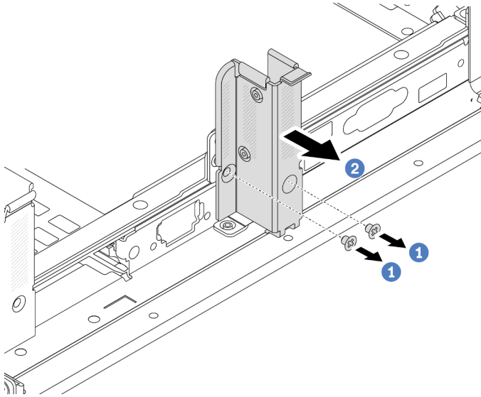
Abbildung 181. Entfernen der Rückwandhalterung B1 (Mitte)
