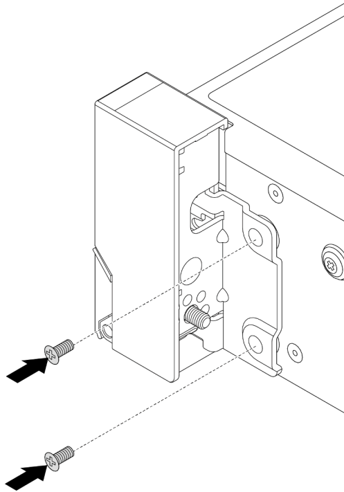
Abbildung 158. Installieren der Schrauben
