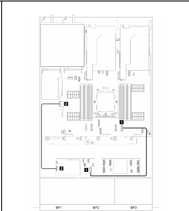
Abbildung 336. Signalkabelführung Teil 2
