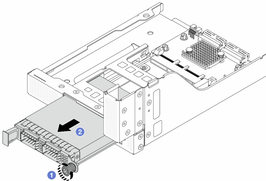
Abbildung 22. Herausnehmen des OCP-Moduls
