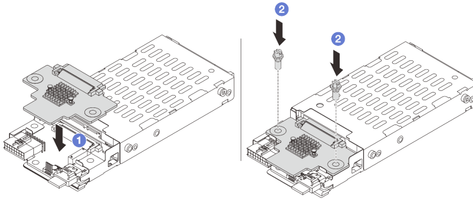
Abbildung 193. Installieren der Rückwandplatten für 7-mm-Laufwerke (oben)
