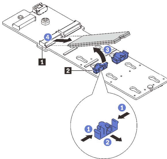
Abbildung 89. M.2-Laufwerk entfernen
