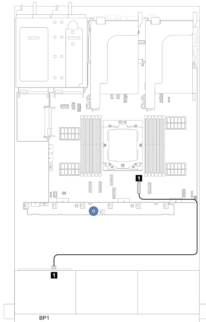
Abbildung 295. SAS/SATA-Kabelführung zu integriertem SATA-Anschluss
