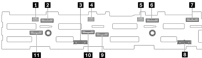
Abbildung 247. Anschlüsse an der 12 x 3,5-Zoll-AnyBay-Rückwandplatine
