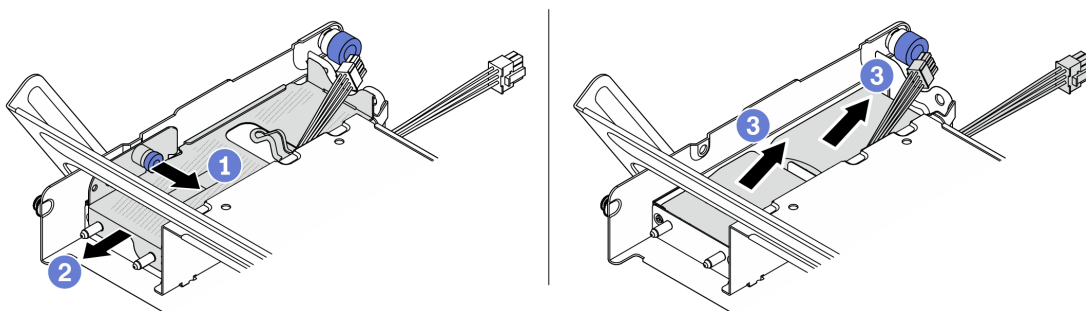
Abbildung 176. RAID-Flash-Stromversorgungsmodul aus der mittleren Laufwerkhalterung entfernen.
