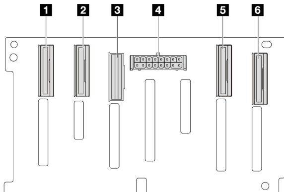
Abbildung 242. Anschlüsse an der 8 x 2,5-Zoll-AnyBay-Rückwandplatine
