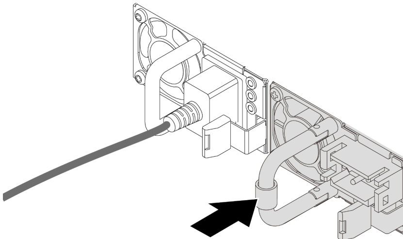
Abbildung 144. Installieren der Netzteilereinheit
