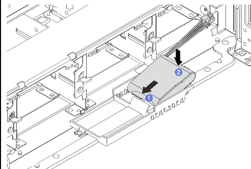
Abbildung 171. Installieren Sie das RAID-Flash-Stromversorgungsmodul auf der Superkondensator-Halterung.
