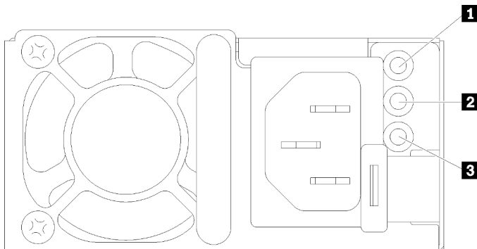
Abbildung 393. Netzteilanzeigen
