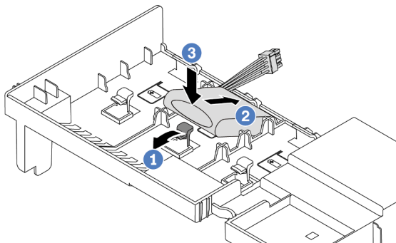
Abbildung 173. Installieren des RAID-Flash-Stromversorgungsmoduls an der Luftführung
