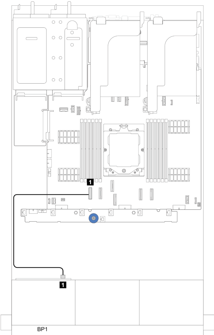
Abbildung 296. Kabelführung mit einem installierten Prozessor
