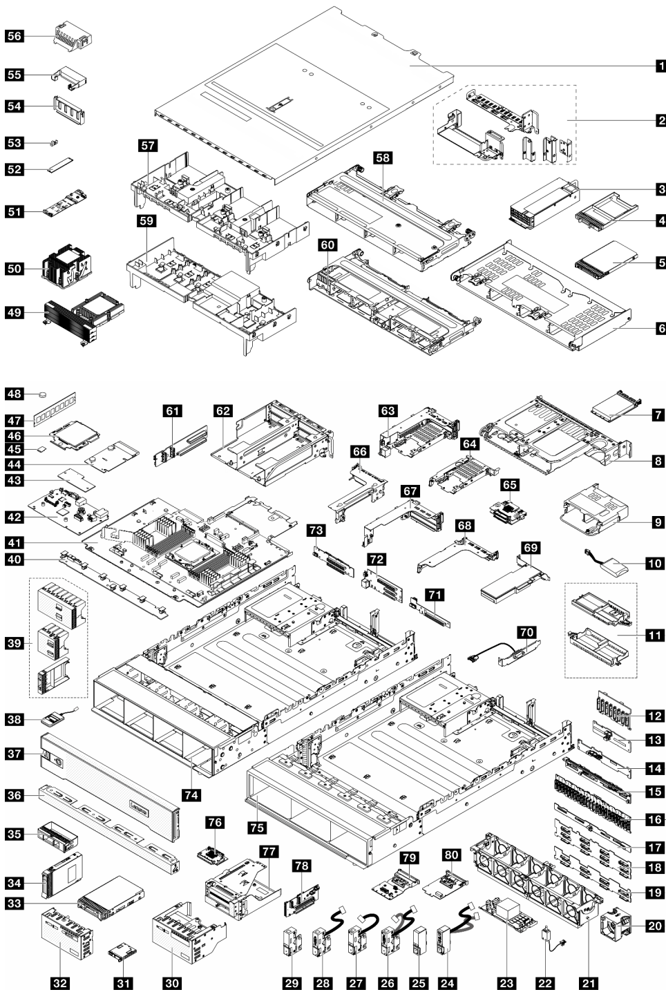
Abbildung 19. Serverkomponenten
