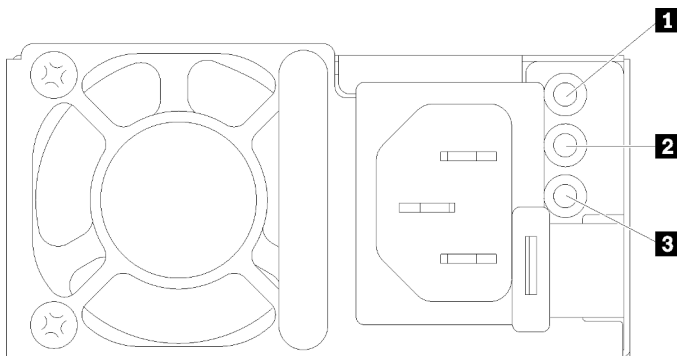
Figura 16. LED dell'alimentatore
