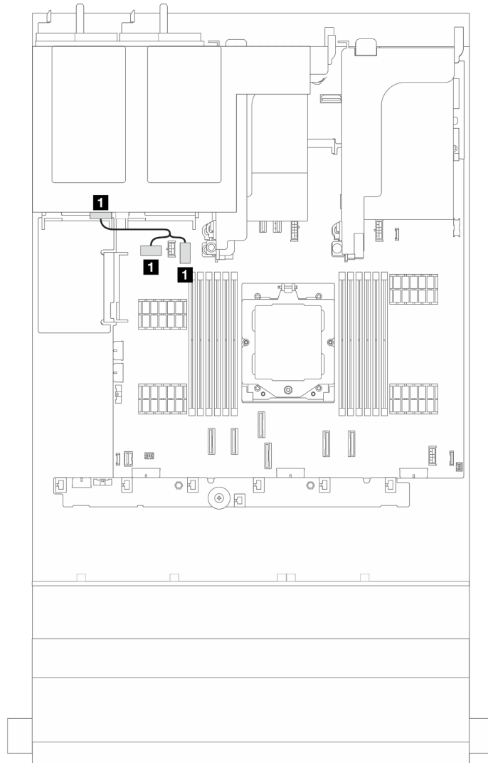
図 289. 背面ドライブ・バックプレーン用電源ケーブル接続
