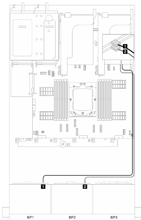
図 318. 信号ケーブルの配線、パート 1
