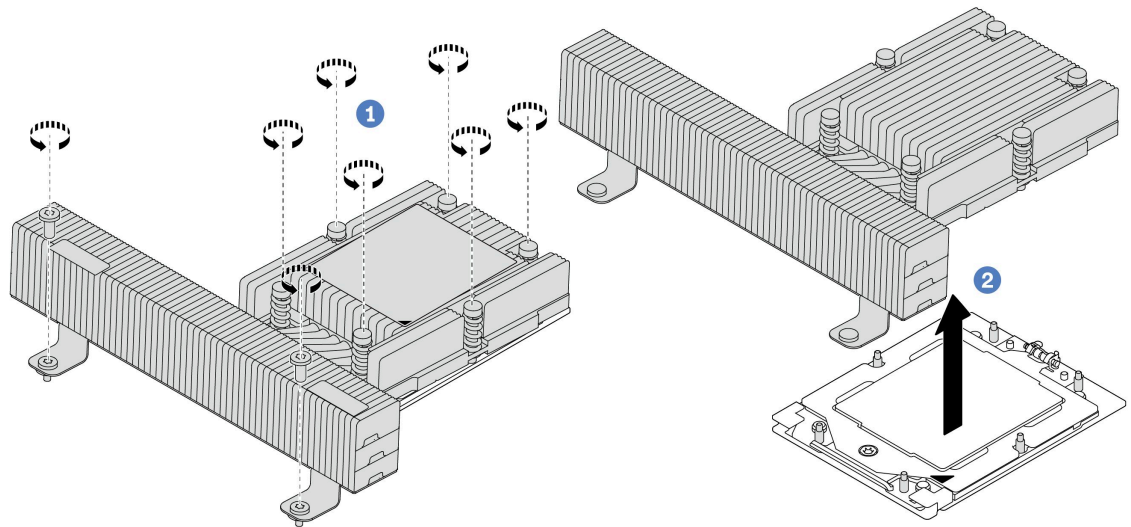
図 147. パフォーマンス・ヒートシンクの取り外し
