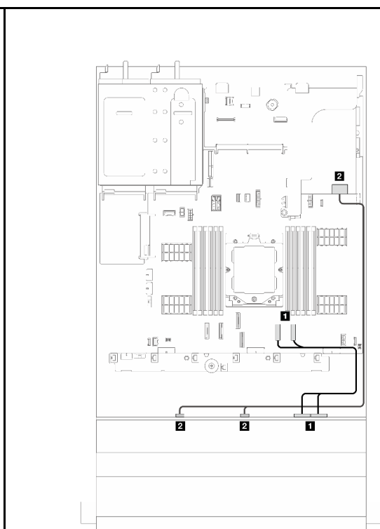
図368. 信号ケーブルの配線 (ライザー 3 対応)
