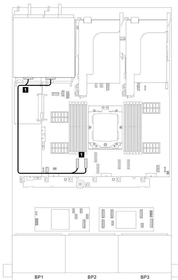
図 328. オンボード・コネクタ用信号ケーブルの配線
