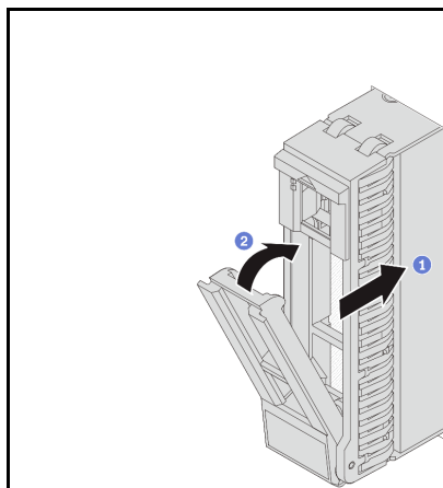
図 81. 2.5 型ホット・スワップ・ドライブ
