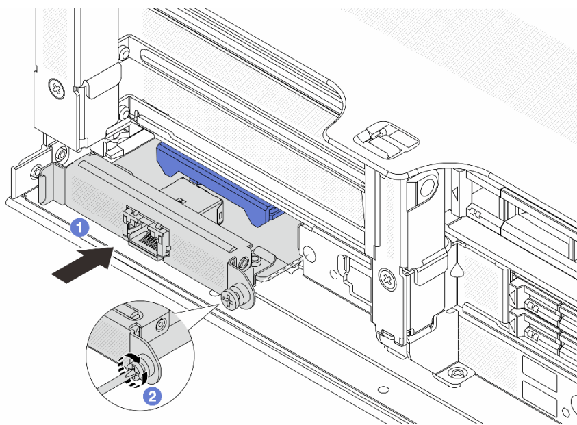
図 104. 管理 NIC アダプターの取り付け
