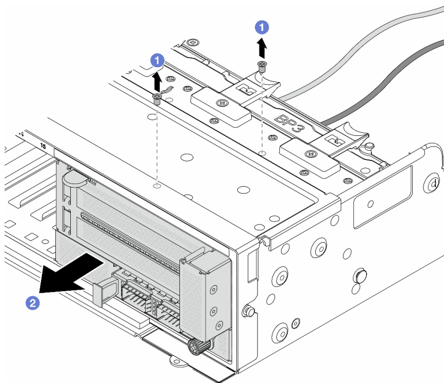
図 18. 前面アダプター・アセンブリーの取り外し
