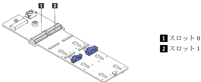
図91. M.2 ドライブ・スロット
