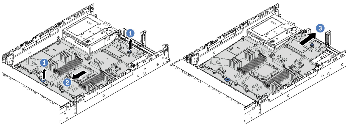
図 223. システム・ボード・アセンブリーの取り外し
