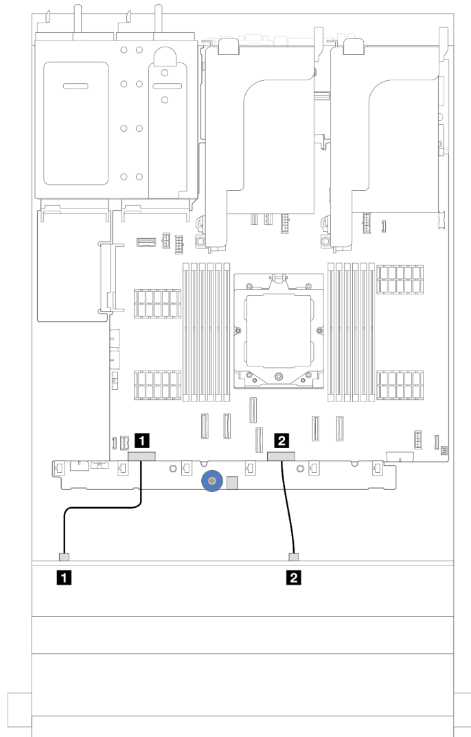
図 358. 12 x 3.5 型 SAS/SATA および AnyBay ドライブ・バックプレーンの電源ケーブルの配線
