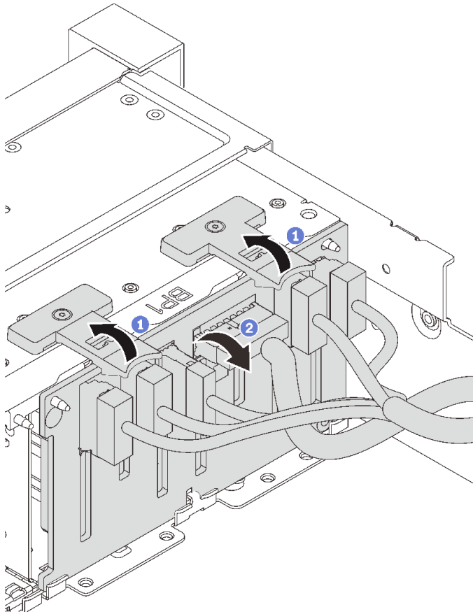
図 52. 2.5 型ドライブ・バックプレーンの取り外し
