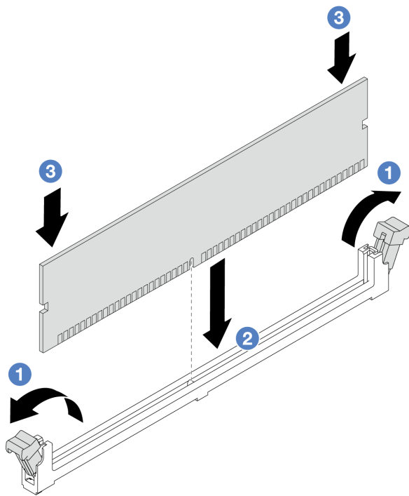
図 106. メモリー・モジュールの取り付け
