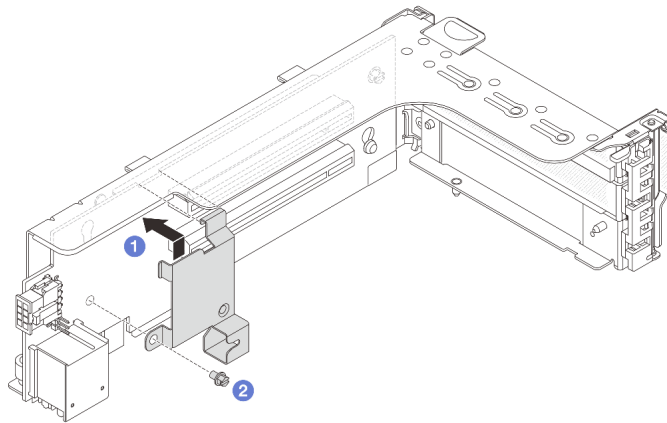
図 194. 7mm ドライブ・ケージの固定クリップの取り付け
