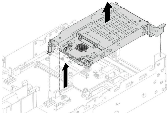
図 187. 7mm SSD ライザー・ケージの取り外し
