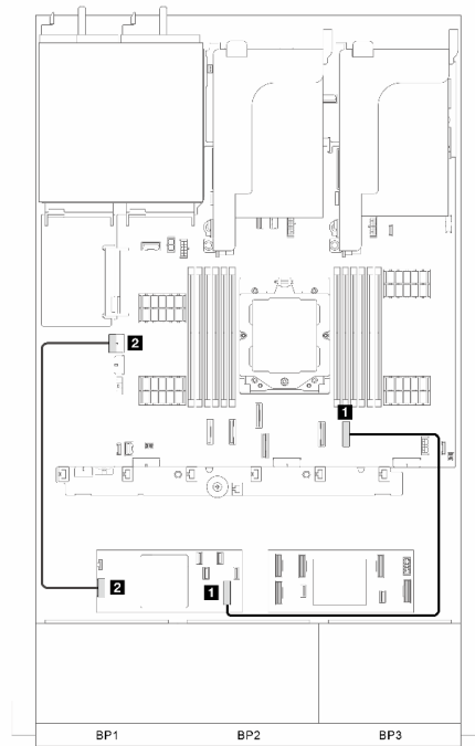
図 330. CFF アダプター用信号ケーブルの配線
