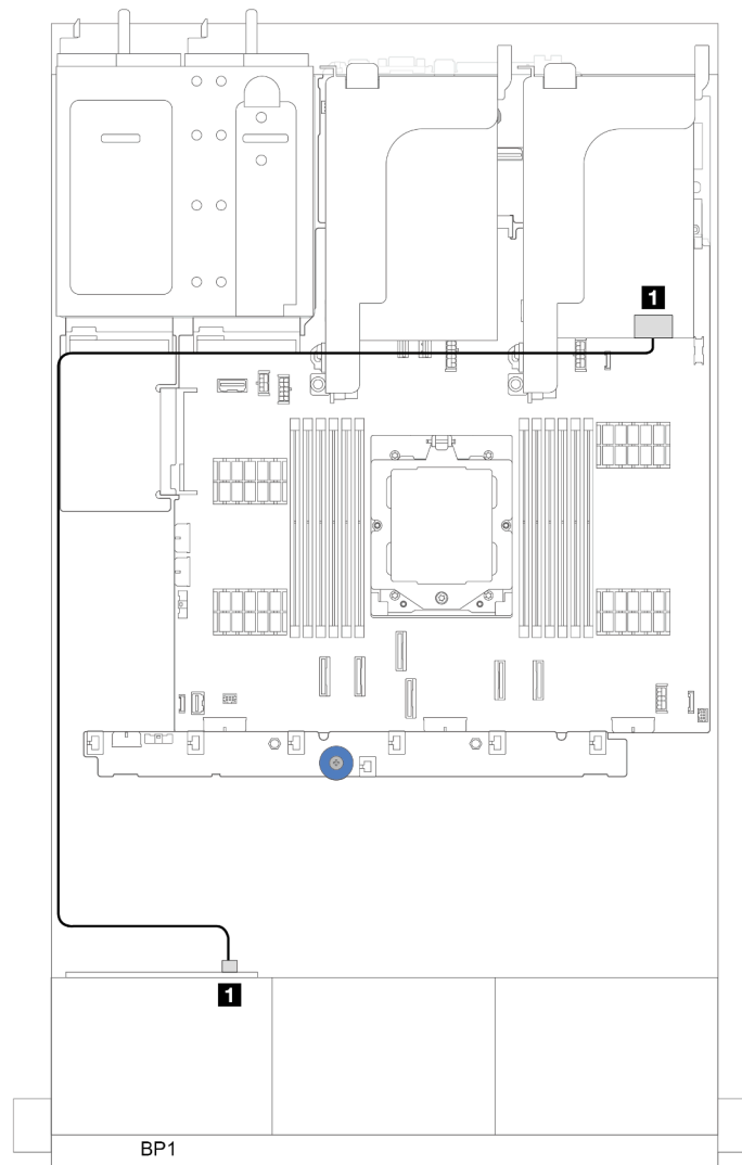
図 293. 8i/16i RAID/HBA アダプターへの SAS/SATA ケーブル配線
