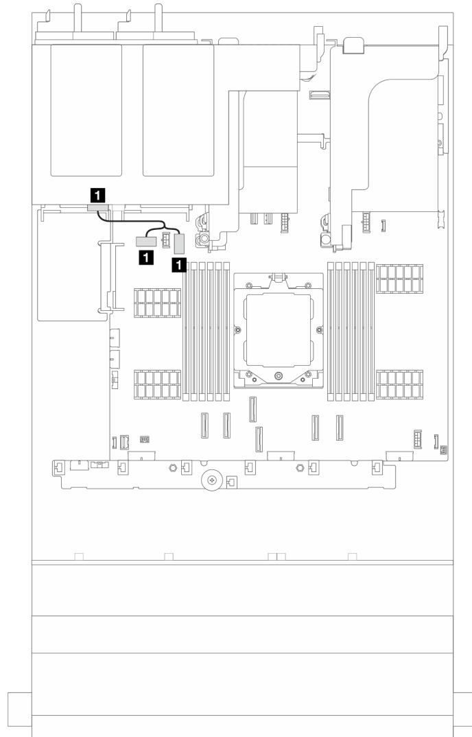
図 360. 2 x 3.5 型 および 4 x 2.5 型 背面ドライブ・バックプレーンの電源ケーブルの配線
