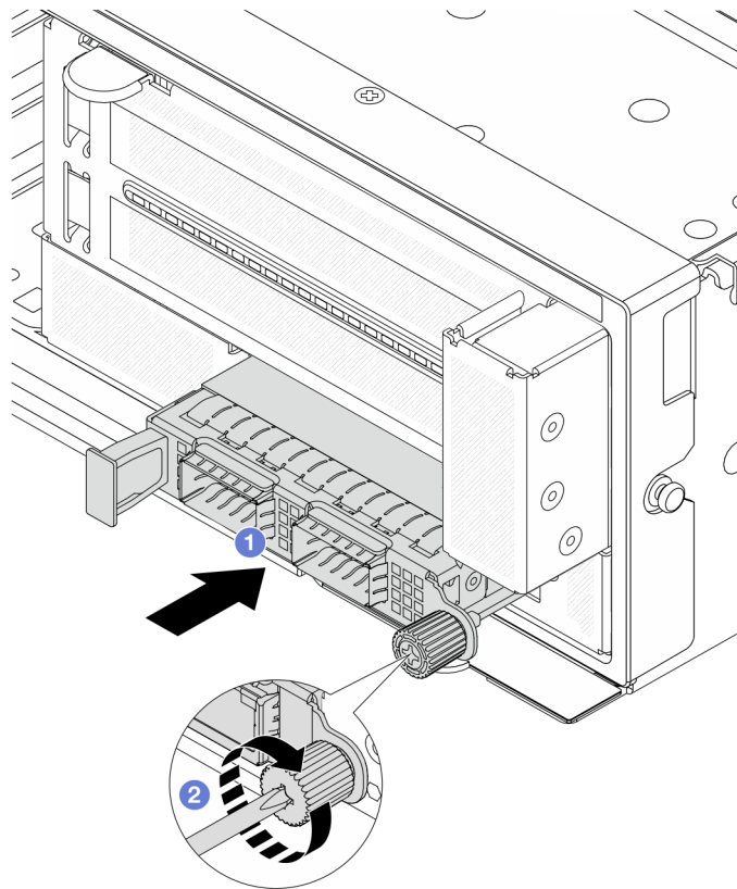
図31. 前面 OCP モジュールの取り付け
