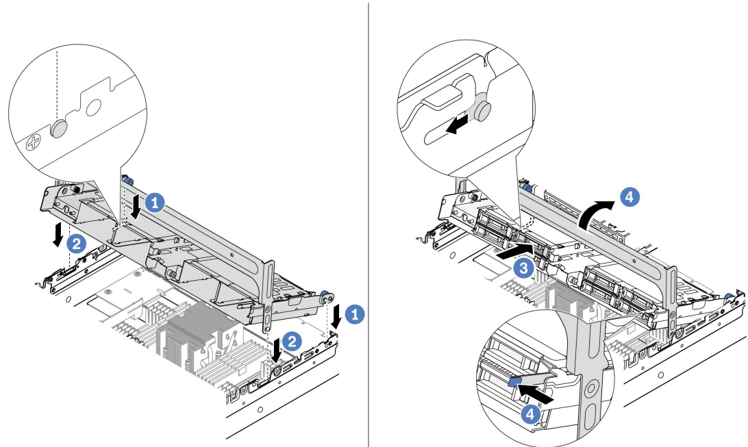
図 114. 中央ドライブ・ケージとドライブの取り付け
