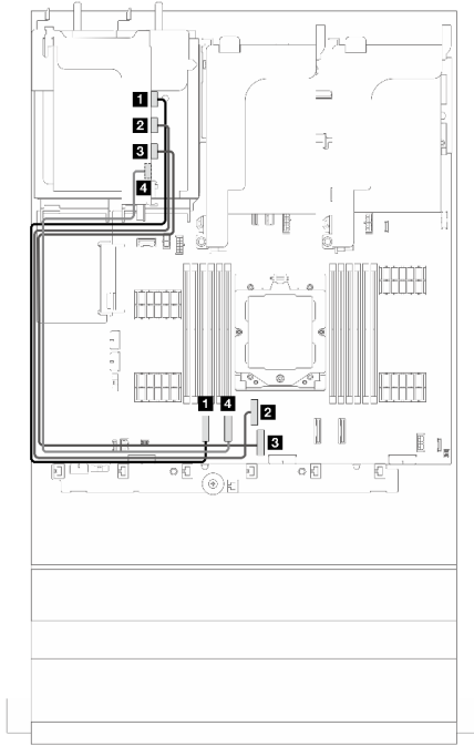
図 280. ライザー 3 (x16/x16 Gen 4) 信号ケーブルの配線
