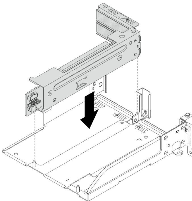
図 134. ライザー 3/4 アセンブリーの取り付け
