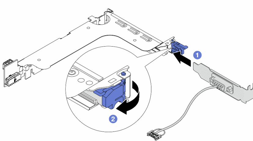
図 236. シリアル・ポート・モジュールの取り付け
