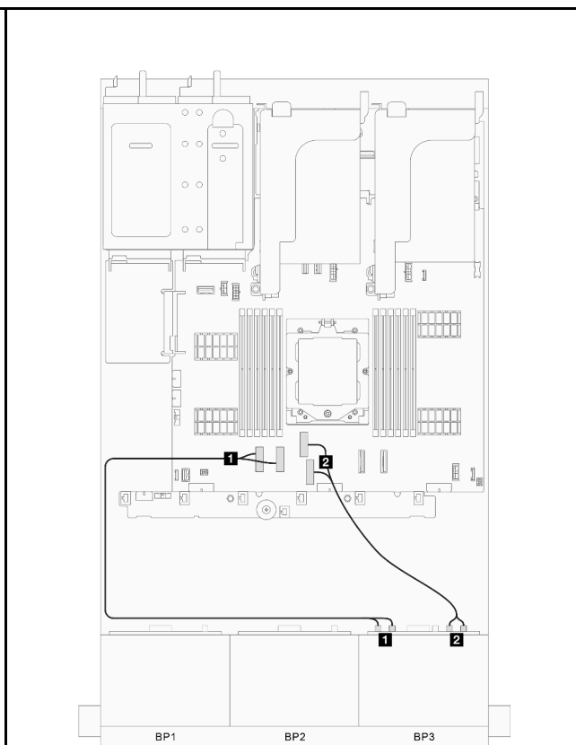
図 315. 信号ケーブルの配線、パート 2
