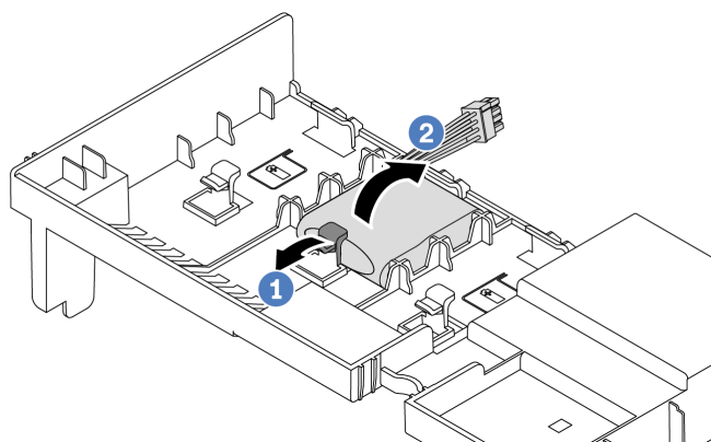
図 172. エアール・バッフルからの RAID フラッシュ電源モジュールの取り外し
