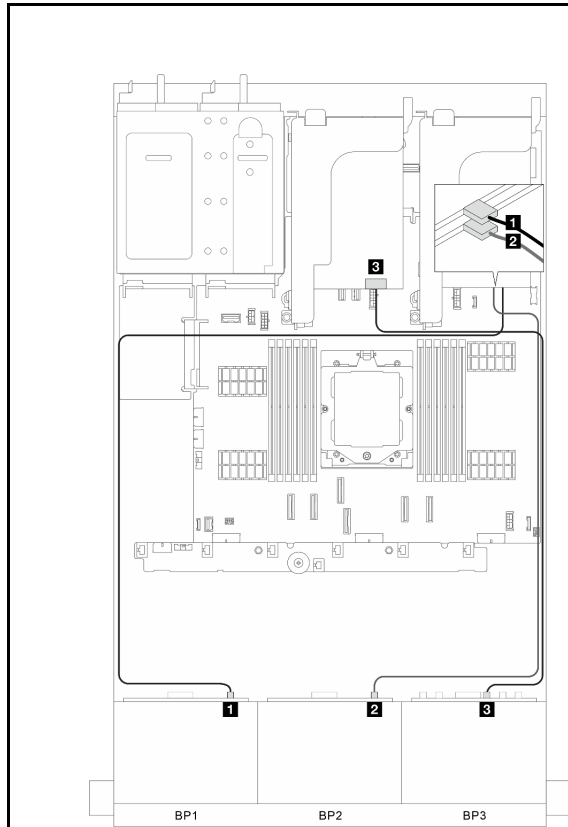
図316. 信号ケーブルの配線、パート 1
