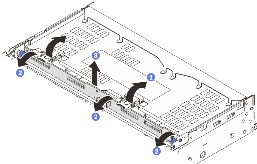
図 211. 4 x 3.5 型背面ドライブ・バックプレーンの取り外し
