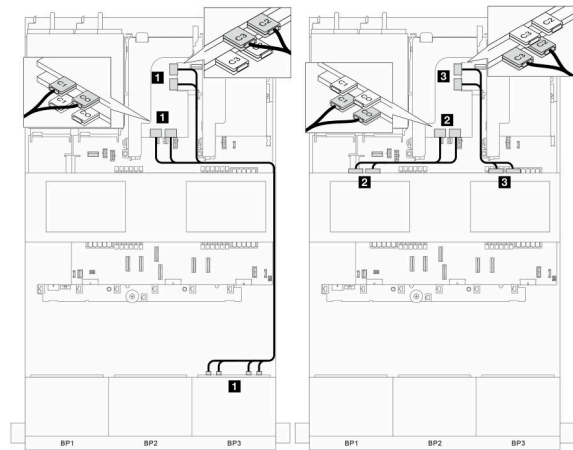
図 352. 信号ケーブルの配線、パート 2
