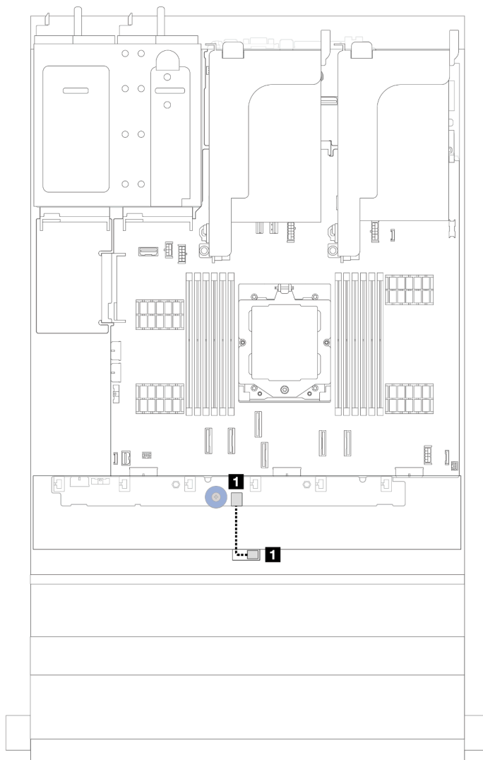
図 264. 侵入検出スイッチ・ケーブルの配線
