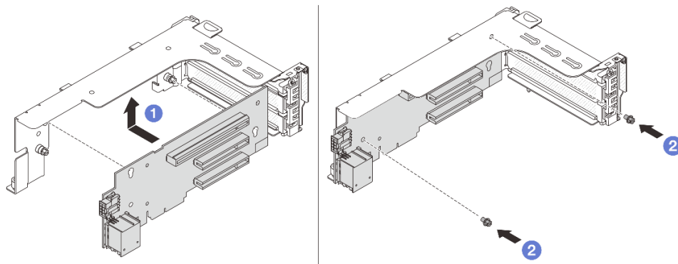
図 125. ライザー・カード 1 の取り付け
