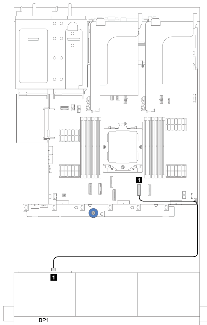
図 295. オンボード SATA コネクタへの SAS/SATA ケーブル配線
