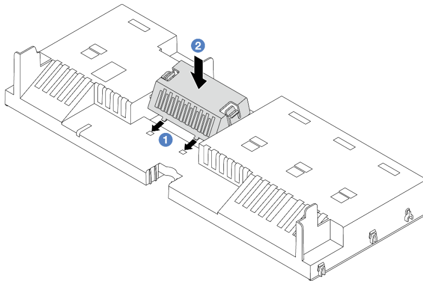
図 14. エア・バッフル・フィルラ-の取り付け
