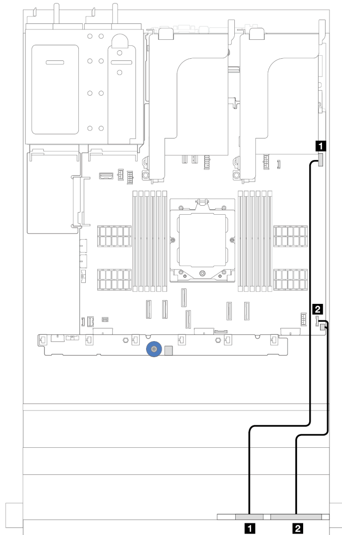
図 262. メディア・ベイ上の内蔵診断パネルのケーブル配線
