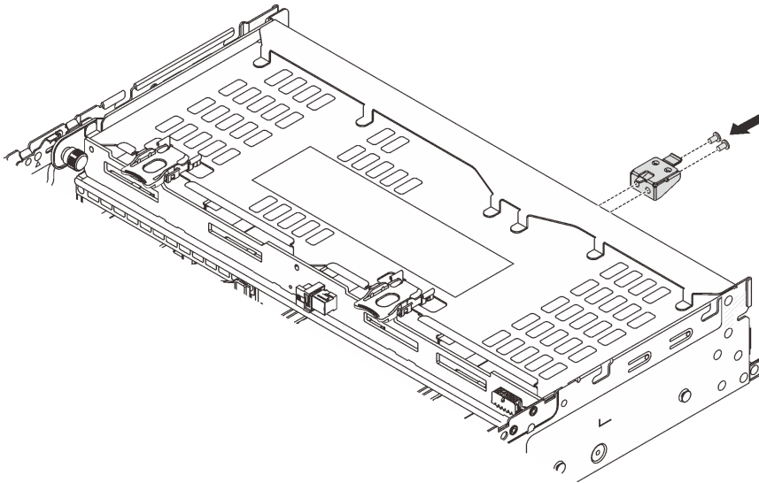
図214. トップ・カバー・サポート・ブラケットの取り付け
