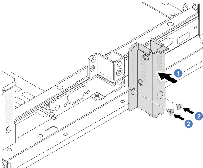
図 184. B1 背面壁ブラケットの取り付け (中央)
