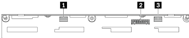
図 252. 8x2.5 型 SAS/SATA バックプレーン・コネクター
