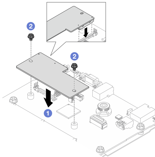
図 222. ファームウェアおよび RoT セキュリティー・モジュールの取り付け
