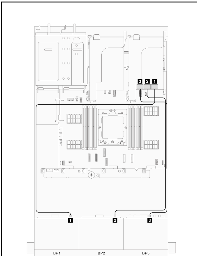
図 310. 信号ケーブルの配線、パート 1
