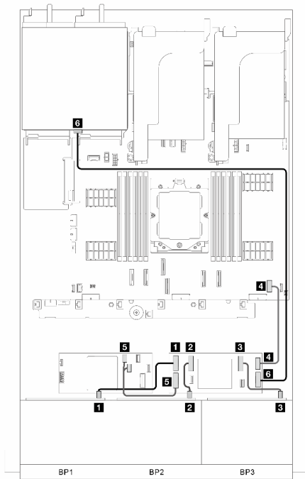
図 329. CFF エクspander用信号ケーブルの配線
