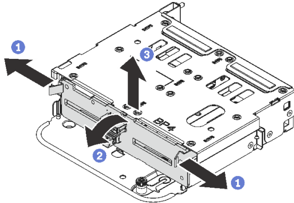
図199. 4 x 2.5 型背面ドライブ・バックプレーンの取り外し
