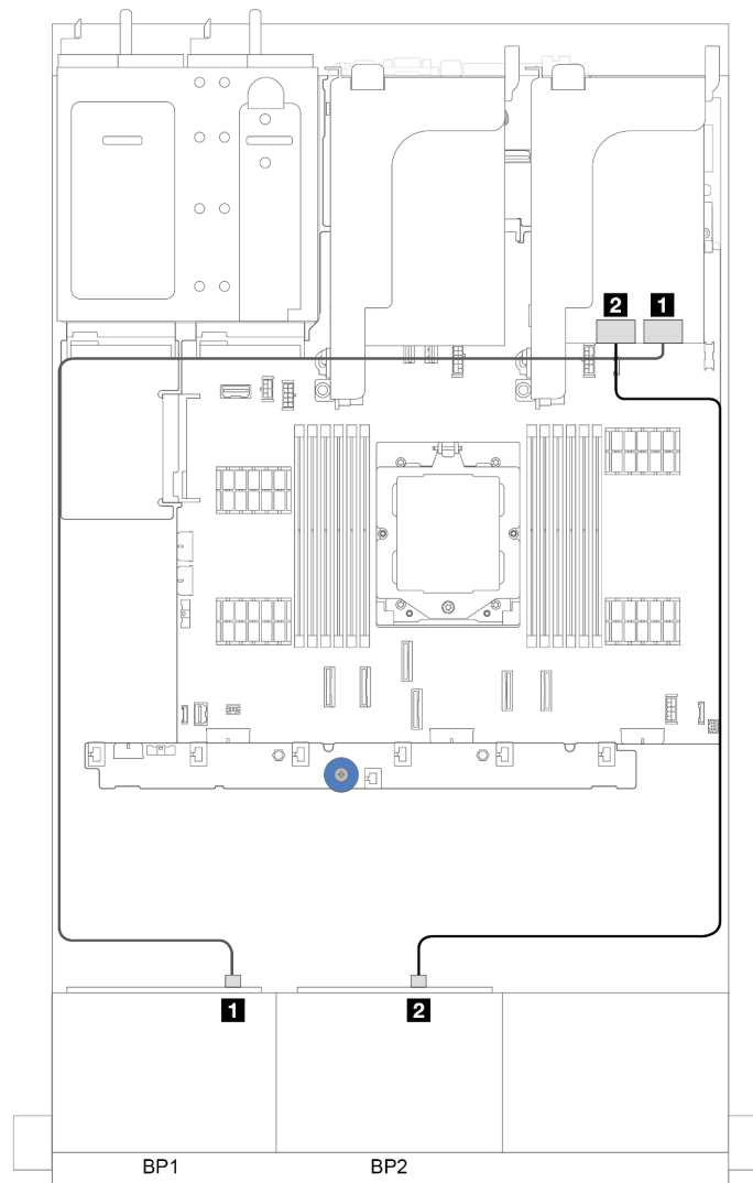
図305. 16i アダプターへの SAS/SATA ケーブル配線
