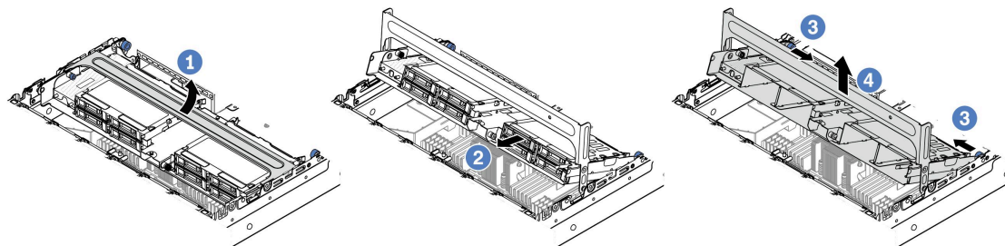
図 109. 中央ドライブ・ケージの取り外し
