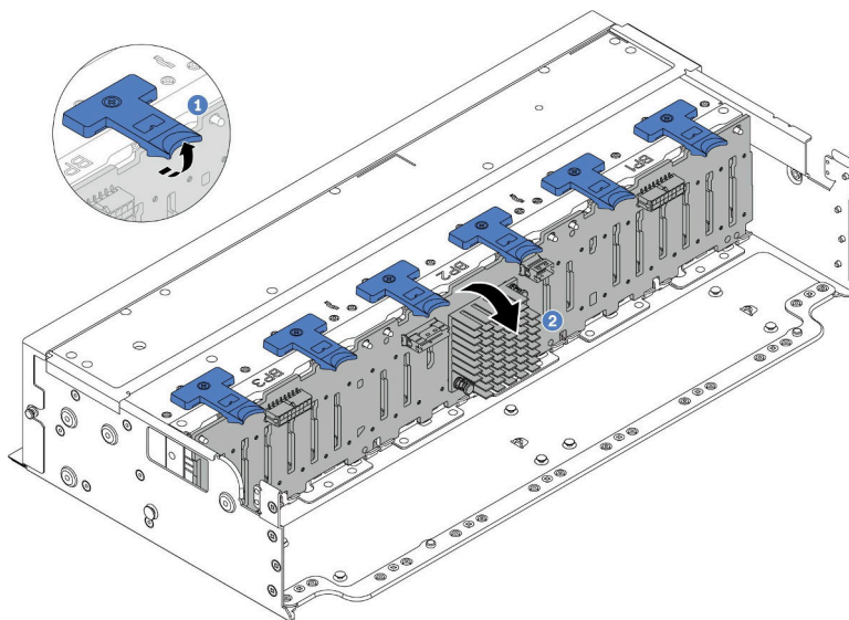
図 53. 24 ベイ・ドライブ・バックプレーンの取り外し
