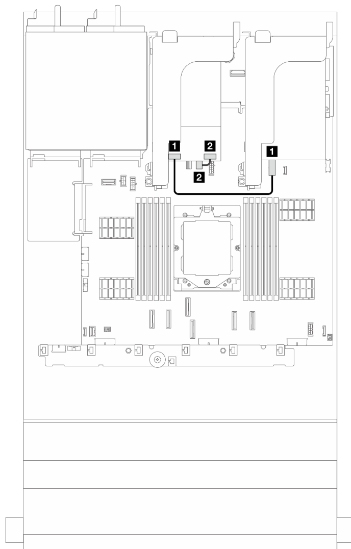
図 256. 7 mm ドライブ・バックプレーン用 NVMe ケーブルの配線
