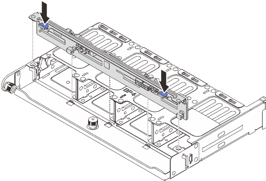
図204. 8 x 2.5 型背面ドライブ・バックプレーンの取り付け
