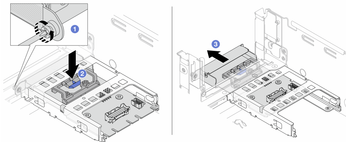
図 40. 背面 OCP 変換コネクタ・カードの取り外し
