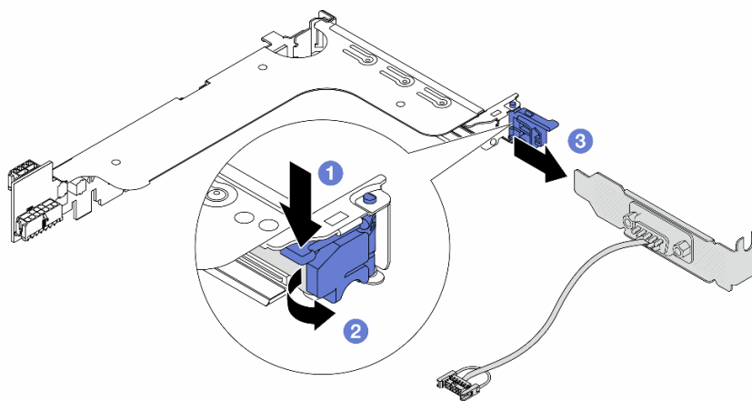
図 233. シリアル・ポート・モジュールの取り外し
