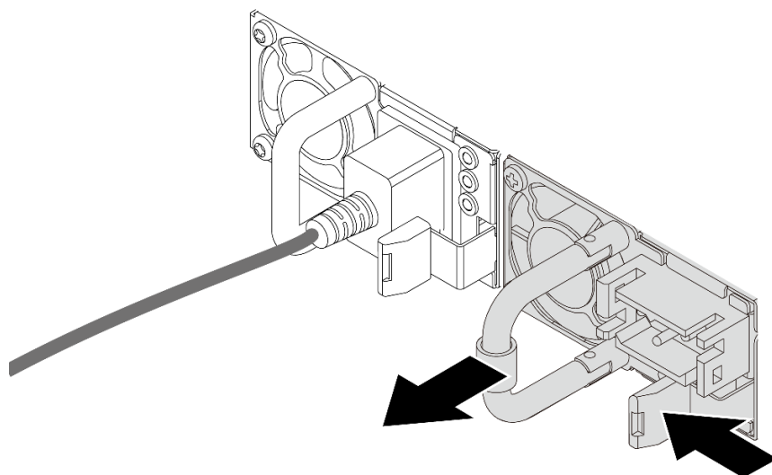
図 142. パワー・サプライ・ユニットの取り外し
