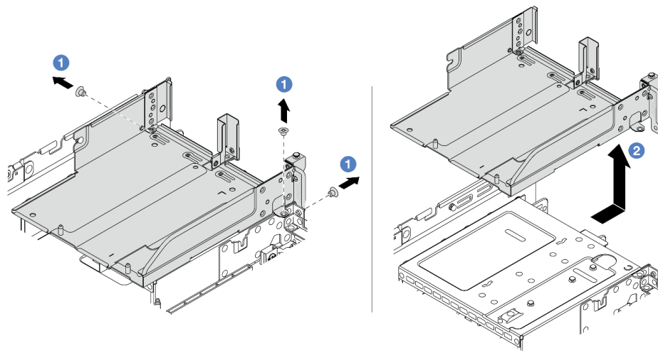
図 118. ライザー・ケージ・トレイの取り外し
