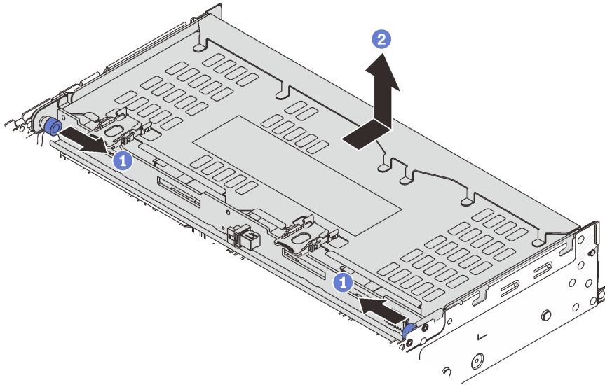
図 210. 4 x 3.5 型背面ドライブ・ケージの取り外し
