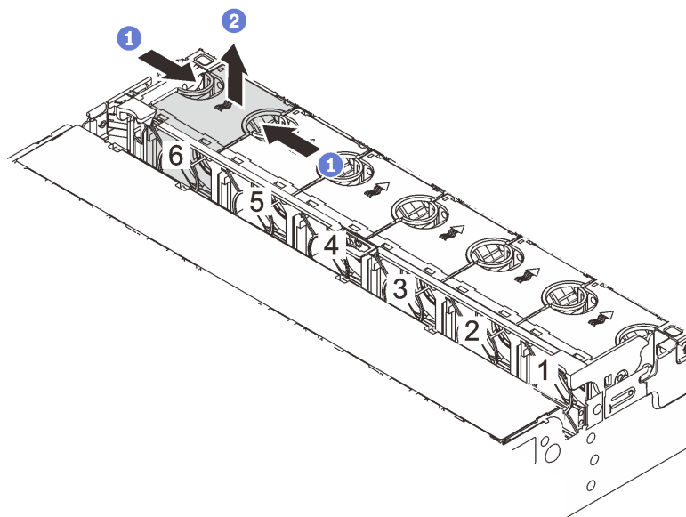
図 227. システム・ファンの取り外し
