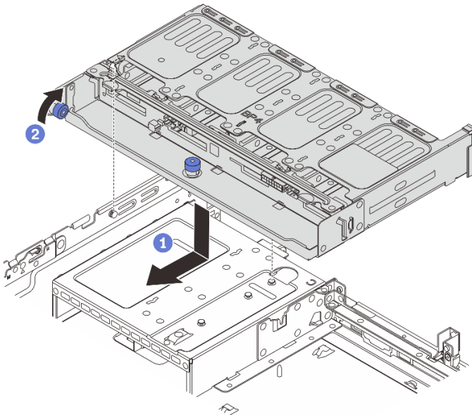
図205. 8 x 2.5 型背面ドライブ・ケージの取り付け
