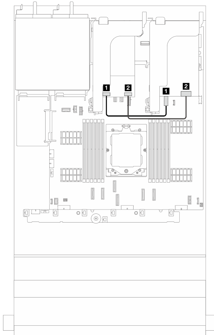
図 257. 7 mm ドライブ・バックプレーン用 RAID ケーブルの配線
