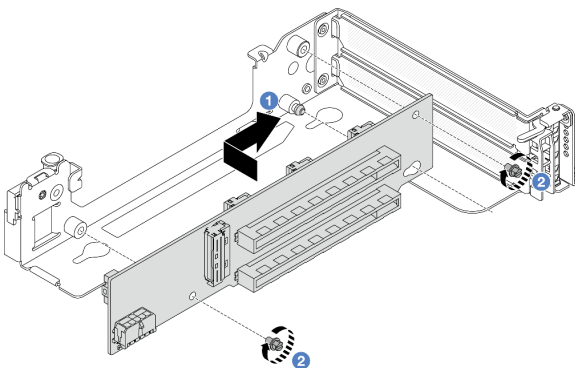
図 126. ライザー・カード 3 の取り付け
