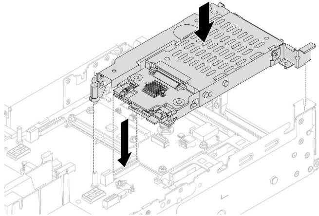
図 197. 7mm SSD ライザー・ケージの取り付け
