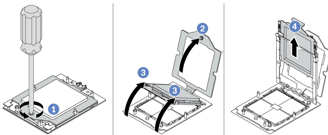
図 148. プロセッサの取り外し
