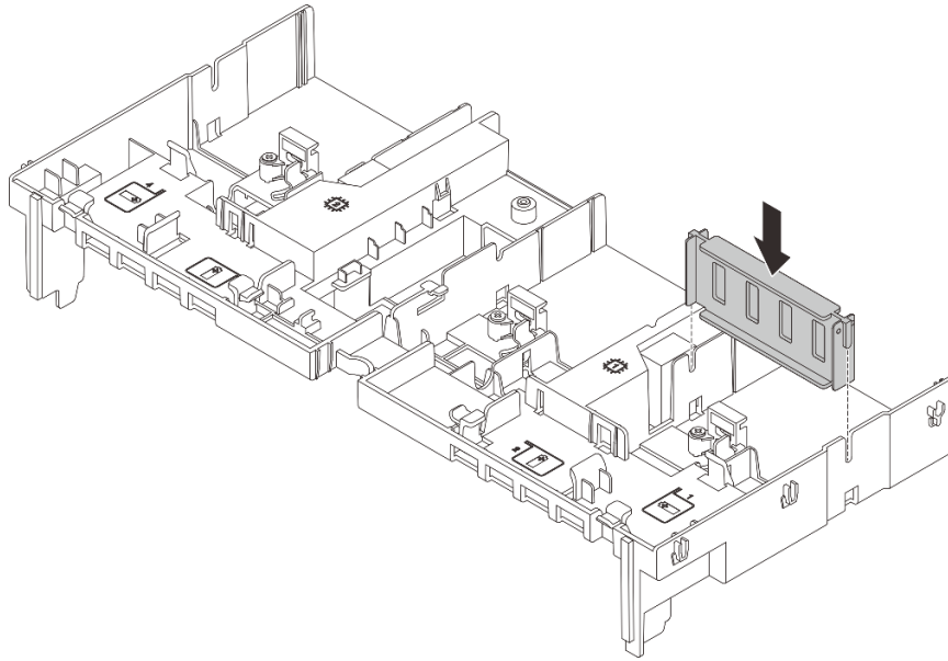
図 76. GPU エアークラップ・フィルターの取り付け
