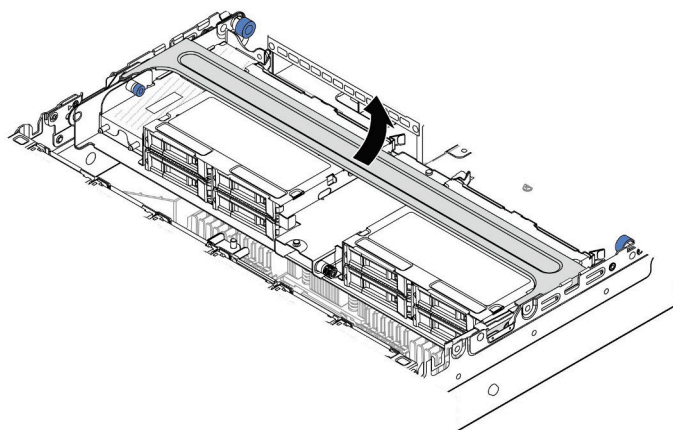
図175. 中央ドライブ・ケージのハンドルを開く
