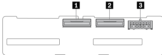
図 249. 4 x 2.5 型 NVMe バックプレーン・コネクター
