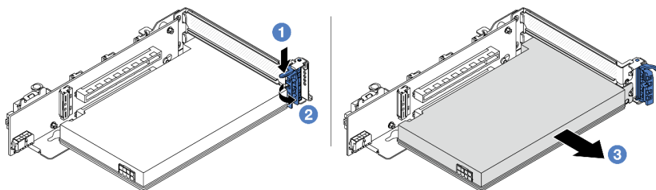
図 120. ライザー 3 アセンブリーからの PCIe アダプターの取り外し
