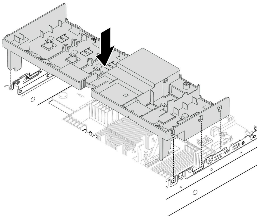
図 15. エアー・バッフルの取り付け
