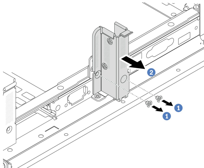
図 181. B1 背面壁ブラケットの取り外し (中央)
