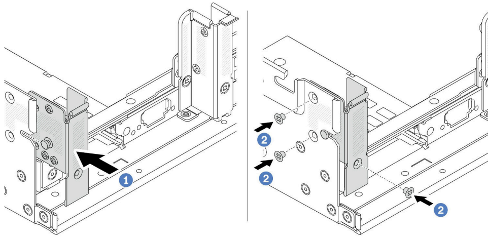
図 183. 左側 A1 背面壁ブラケットの取り付け (左)
