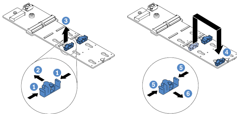
図 90. M.2 保持器具の調整
