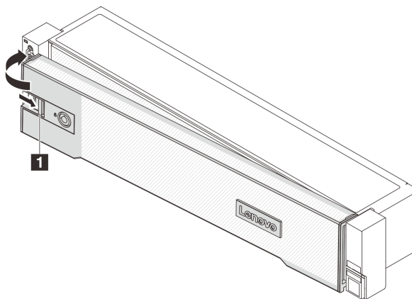
図218. セキュリティー・ベゼルの取り付け
