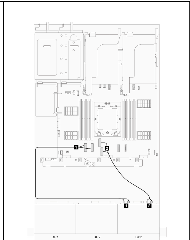
図313. 信号ケーブルの配線、パート 2
