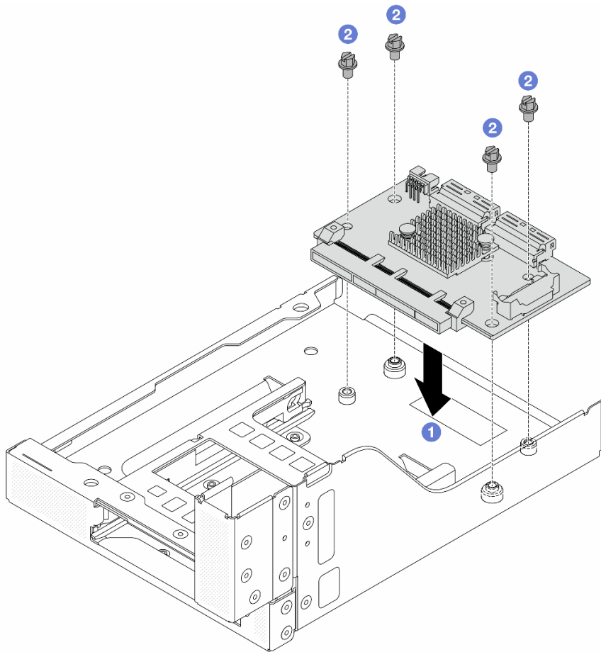
図 24. 前面 OCP 変換コネクタ・カードの取り付け
