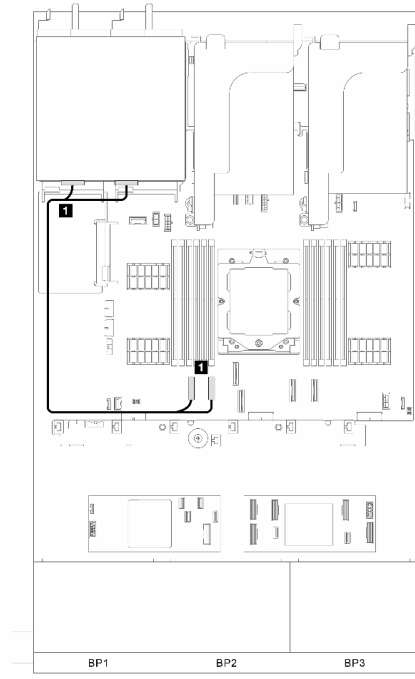
図332. 信号ケーブルの配線、パート 2
