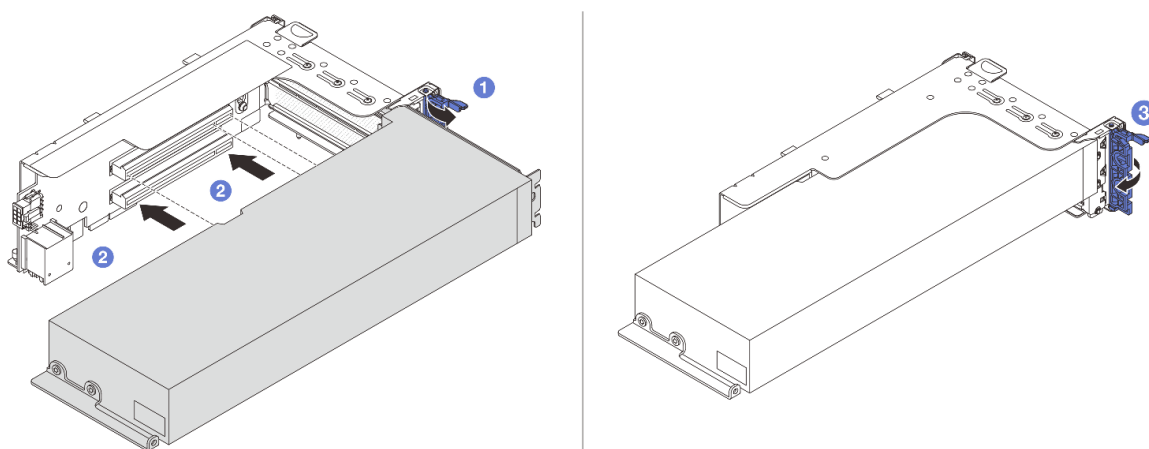
図 73. GPU アダプターの取り付け
