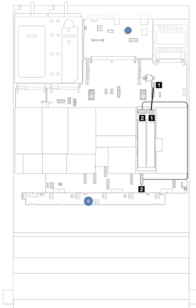
図 268. M.2 ドライブ・バックプレーンの SATA/NVMe ケーブル配線
