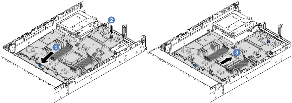
図 226. システム・ボード・アセンブリーの取り付け
