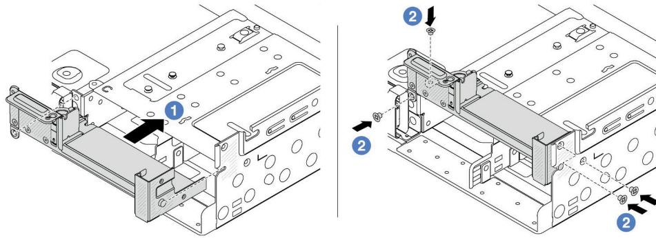
図 185. 左側 C1 背面壁ブラケットの取り付け (右)
