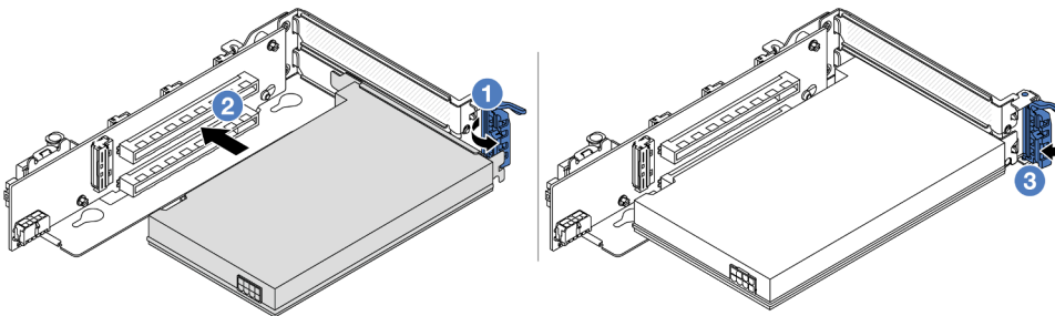
図 129. PCIe アダプターのライザー 3 アセンブリーへの取り付け
