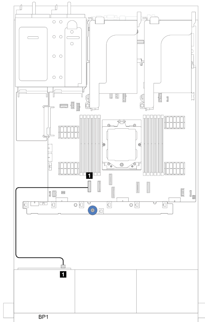
図 296. 1つのプロセッサが取り付けられた場合のケーブル配線
