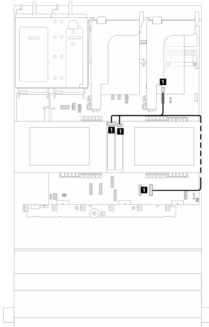
図 266. M.2 ドライブ・バックプレーンの SATA ケーブル配線
