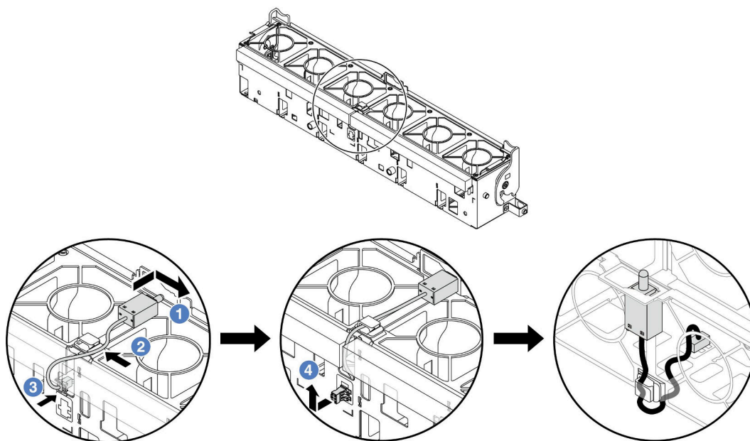
図 88. 侵入検出スイッチの取り付け
