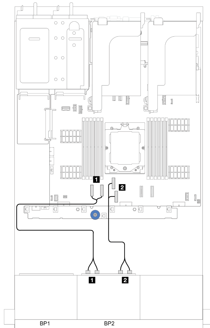
図 306. オンボード・コネクタへの NVMe ケーブル配線
