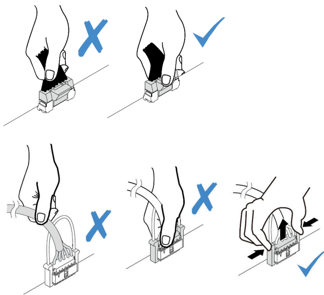
図 83. ケーブルのシステム・ボード・アセンブリーからの切り離し
