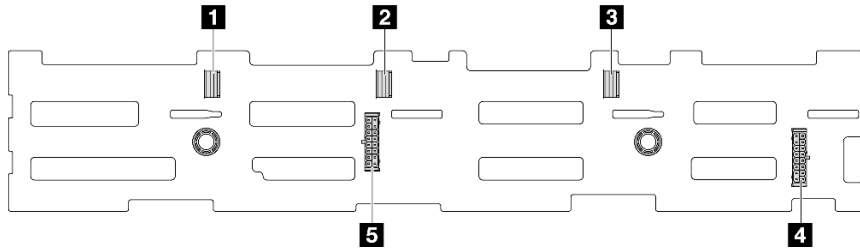
図 245. 12 個の 3.5 型 SAS/SATA バックプレーン・コネクター
