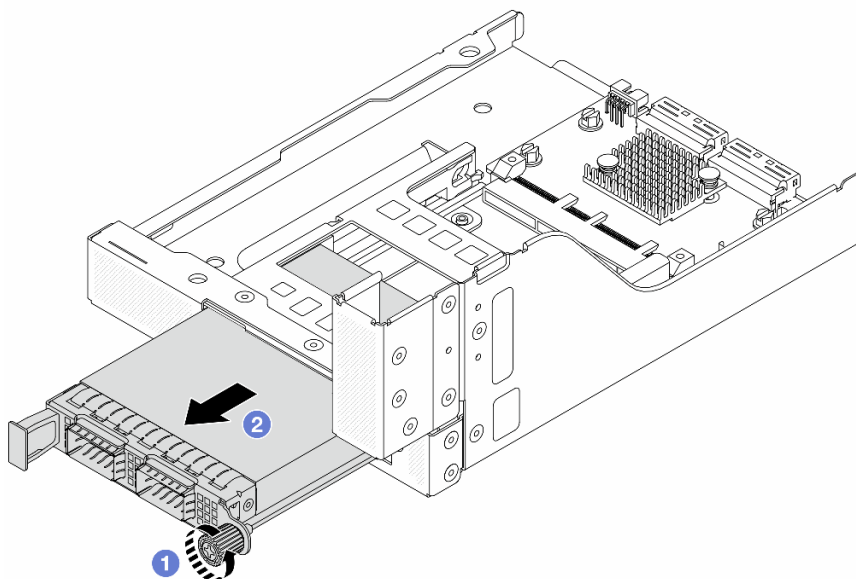
図 22. OCP モジュールの取り外し
