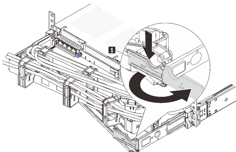
図 141. CMA の調整
