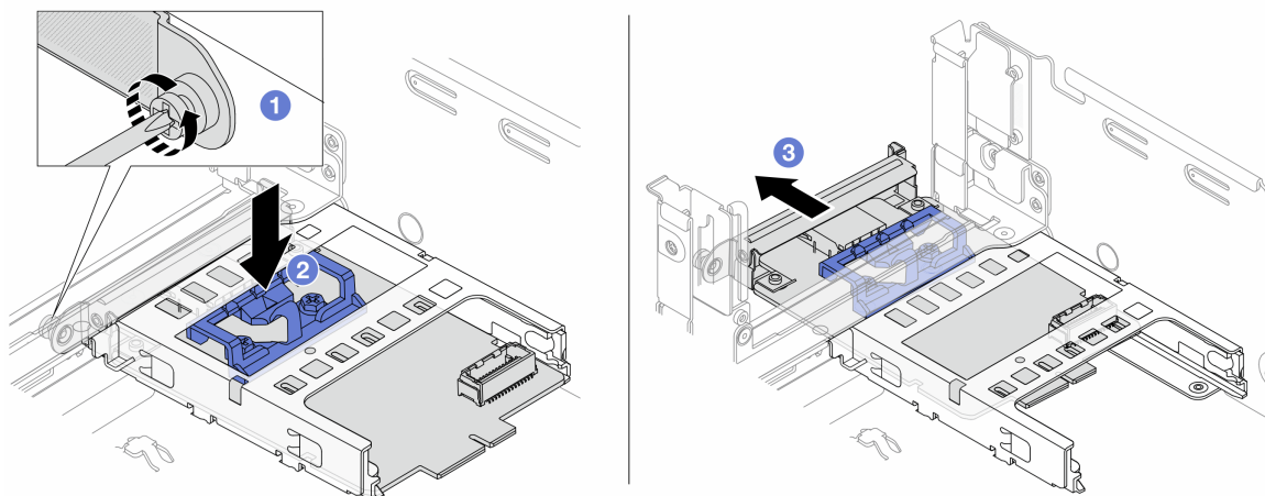
図 103. 管理 NIC アダプターの取り外し
