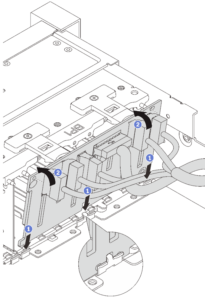
図 55. 2.5 型ドライブ・バックプレーンの取り付け
