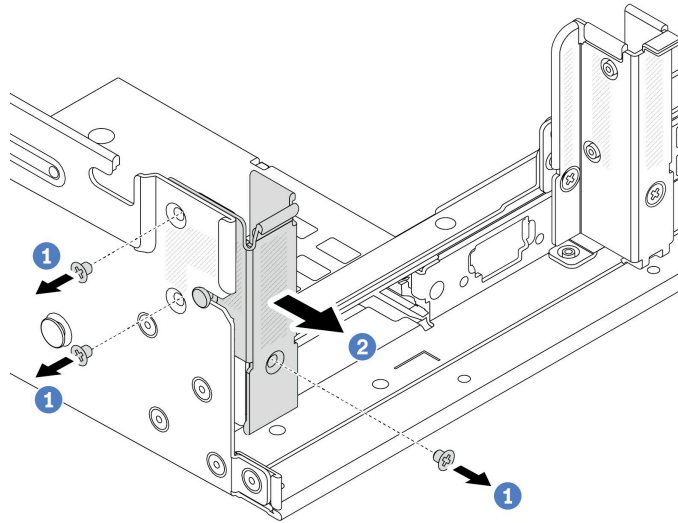
図 180. A1 背面壁ブラケットの取り外し (左)
