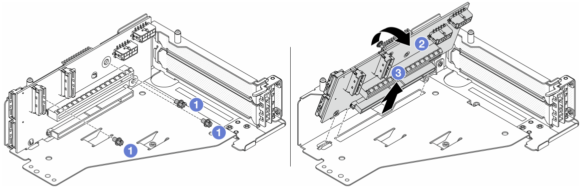
図 45. ライザー 5 ケージからのライザー・カードの取り外し
