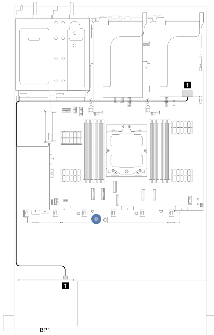
図 291. 8i/16i RAID/HBA アダプターへの SAS/SATA ケーブル配線
