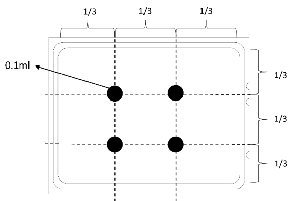
図 150. 熱伝導グリースの塗布
