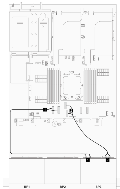
図 319. 信号ケーブルの配線、パート 2
