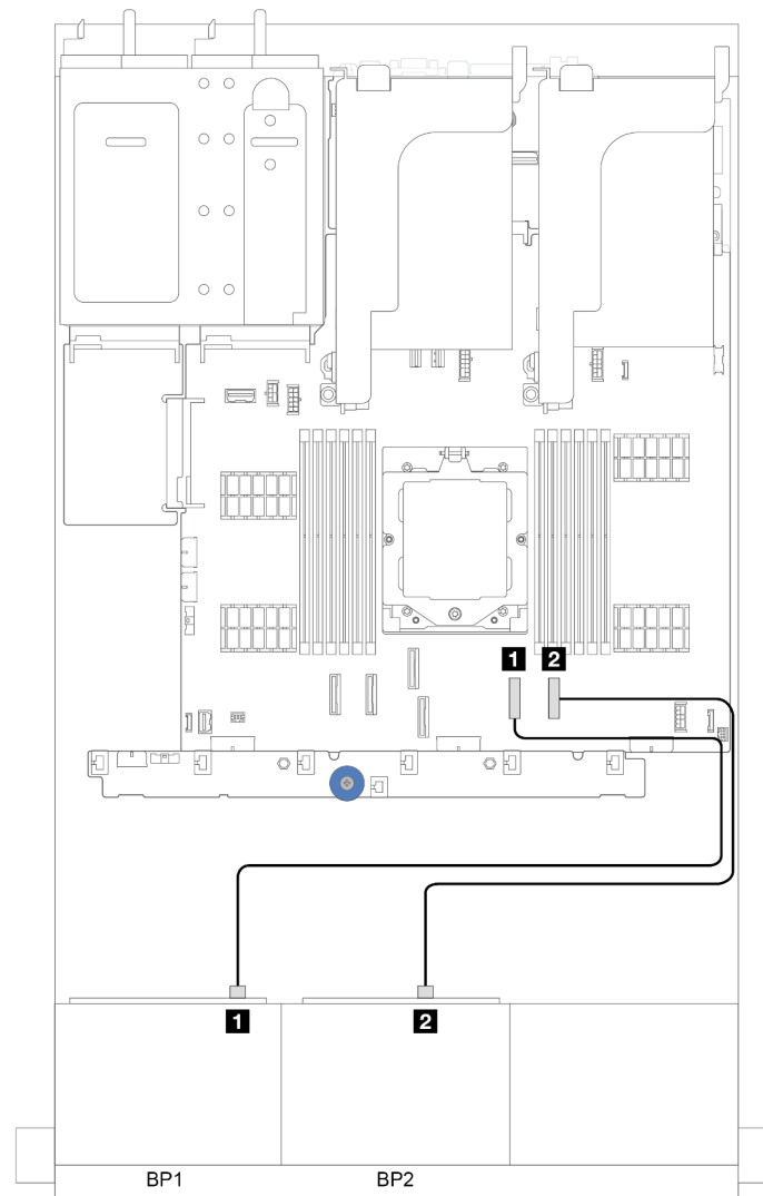
図303. オンボード・コネクタへの SAS/SATA ケーブル配線
