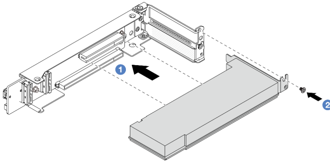
図 130. PCIe アダプターの 4LP ライザー 3/4 アセンブリーへの取り付け
