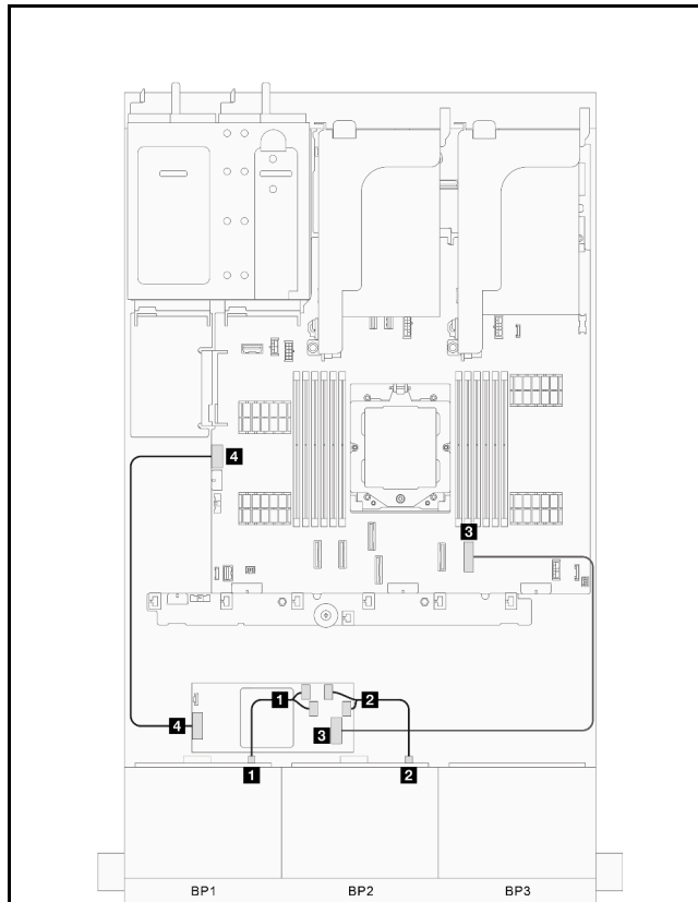
図312. 信号ケーブルの配線、パート 1
