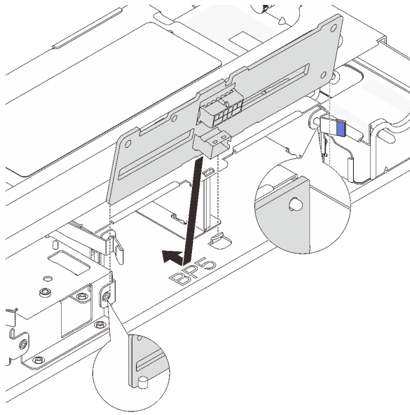
図112. 中央 2.5 型ドライブ・ケージの取り付け
