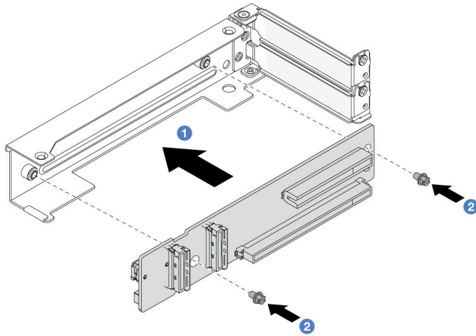
図 127. 4LP ライザー 3/4 ケージへのライザー・カードの取り付け
