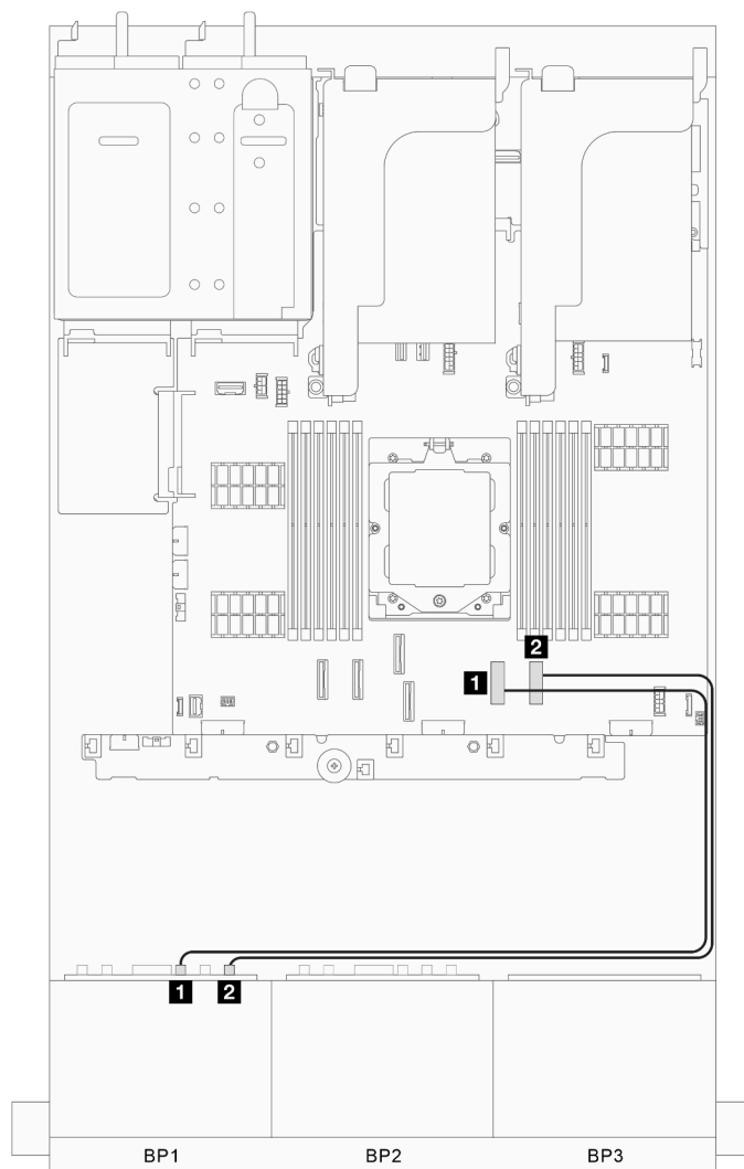
図 297. オンボード・コネクタ (ライザー 3 に対応)
