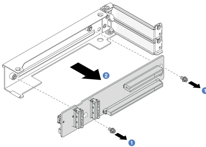
図 124. 4LP ライザー 3/4 ケージからのライザー・カードの取り外し
