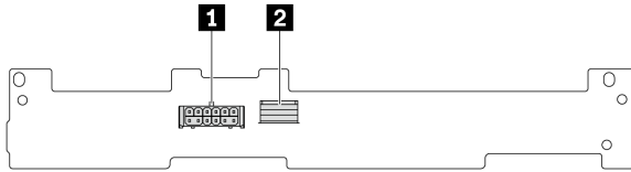
図 251. 2 x 3.5 型 SAS/SATA バックプレーン・コネクター
