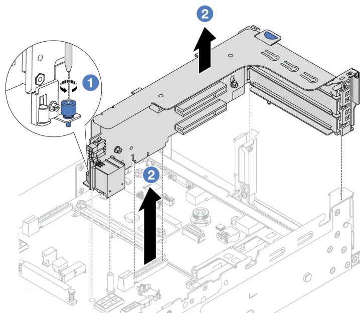
図 115. ライザー・アセンブリー 1 の取り外し
