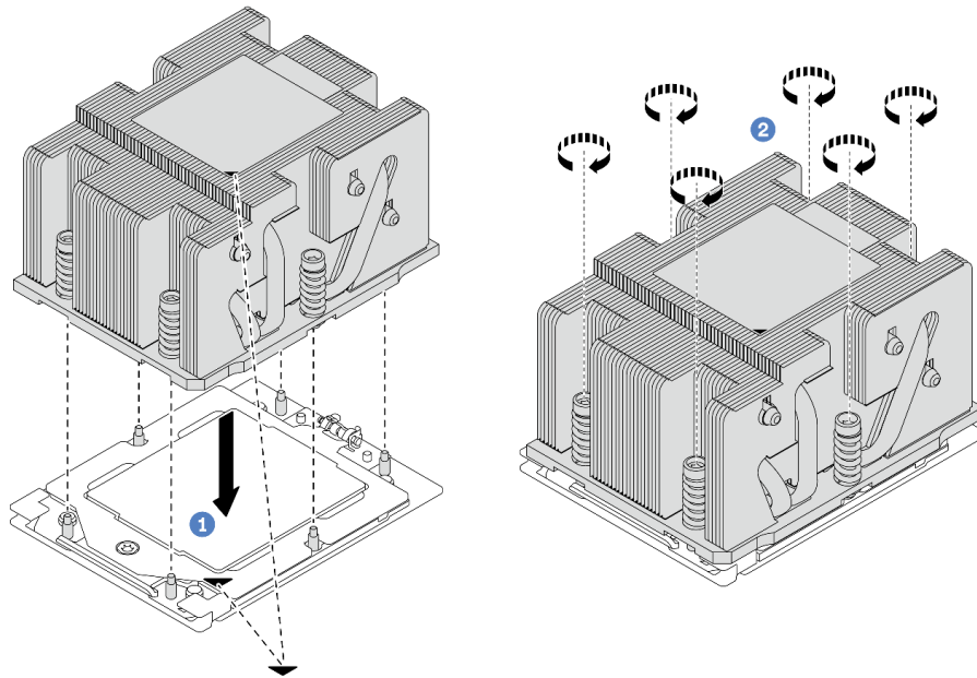
図 151. 標準ヒートシンクの取り付け
