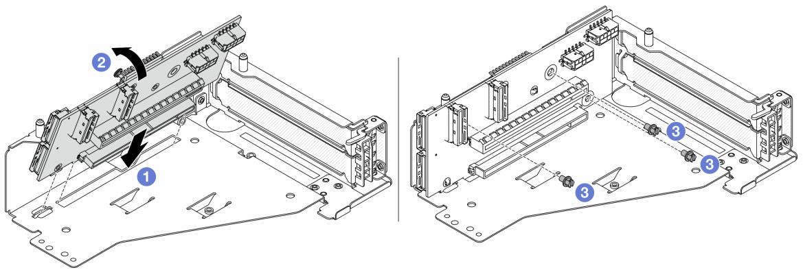
図 26. ライザー・カードの取り付け
