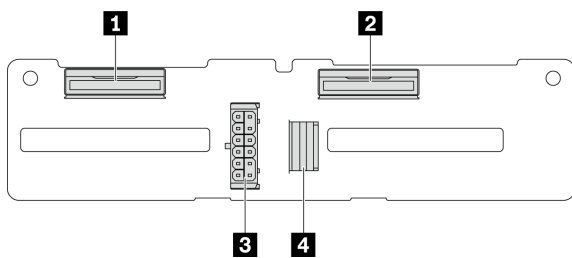
図 253. 4 x 2.5 型 AnyBay バックプレーン・コネクター
