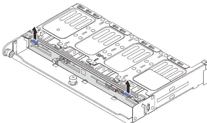
図 203. 背面 8 x 2.5 型ドライブ・バックプレーンの取り外し
