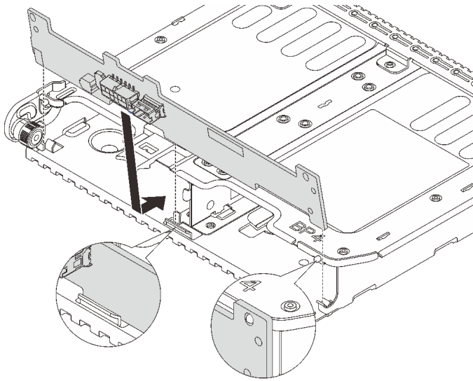
図208. 2 x 3.5 型背面ドライブ・バックプレーンの取り付け
