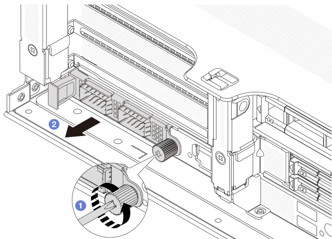
図 135. 背面 OCP モジュールの取り外し
