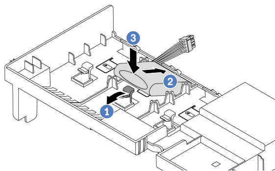
図 173. エアー・バッフルへの RAID フラッシュ電源モジュールの取り付け
