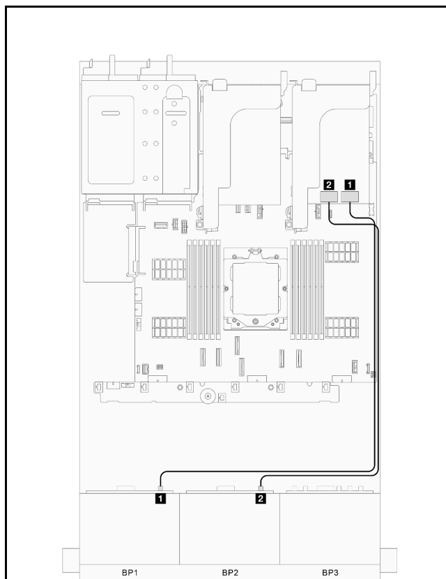
図 314. 信号ケーブルの配線、パート 1
