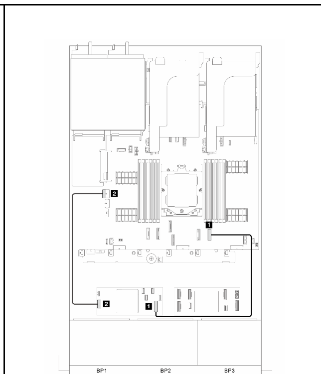
図 336. 信号ケーブルの配線、パート 2
