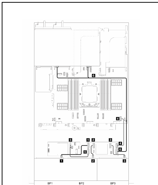
図 335. 信号ケーブルの配線、パート 1
