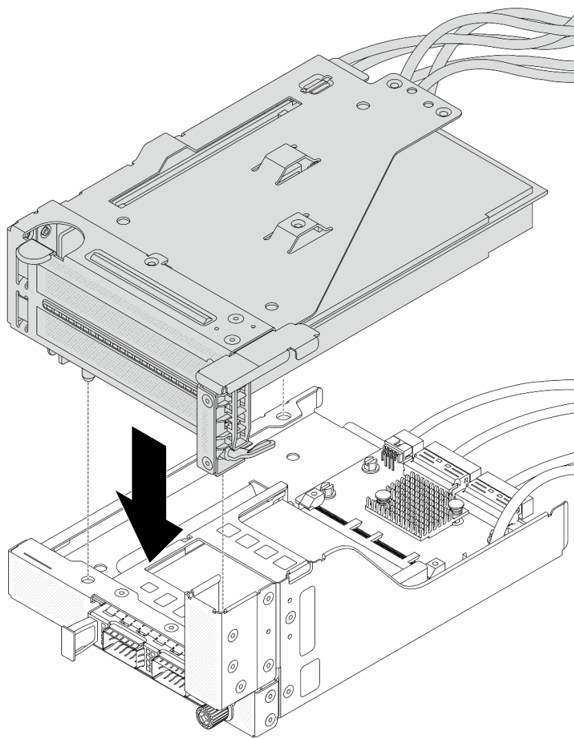
図28. ライザー 5 アセンブリーの前面 OCP アセンブリへの取り付け
