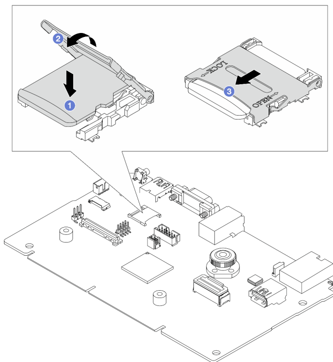
図 108. MicroSD カードの取り付け
