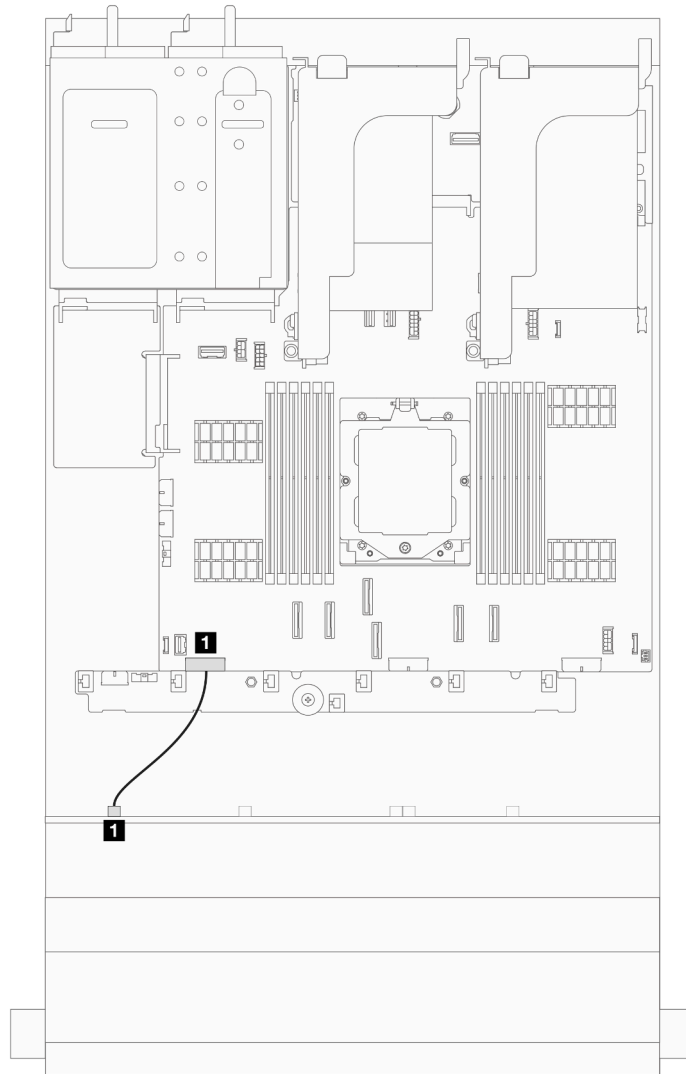
図 359. 12 x 3.5 型 SAS/SATA エクスパンダー前面ドライブ・バックプレーンの電源ケーブルの配線
