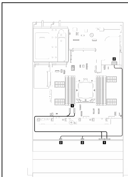
図367. 信号ケーブル配線
