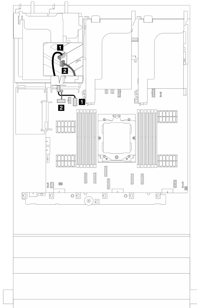
図 277. ライザー 3 電源および側波帯接続 (Gen4/Gen5)
