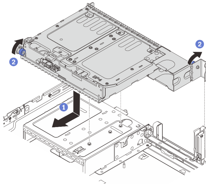
図209. 2 x 3.5 型背面ドライブ・ケージの取り付け
