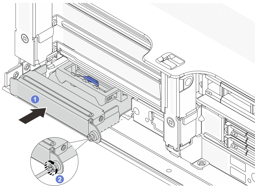
図 41. 背面 OCP 変換コネクタ・カードの取り付け
