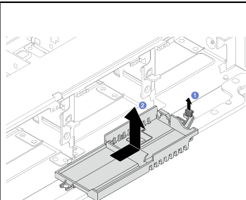
図 167. スーパーキャップ・ホルダーの取り外し
