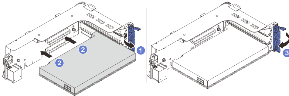
図 128. PCIe アダプターのライザー 1 または 2 アセンブリーへの取り付け
