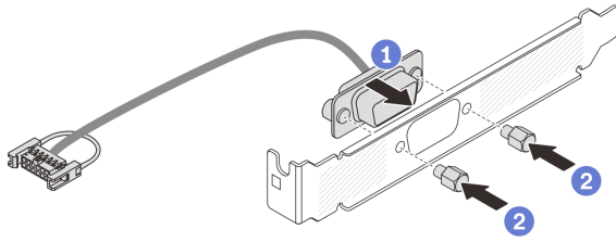
図 235. シリアル・ポート・モジュールの組み立て
