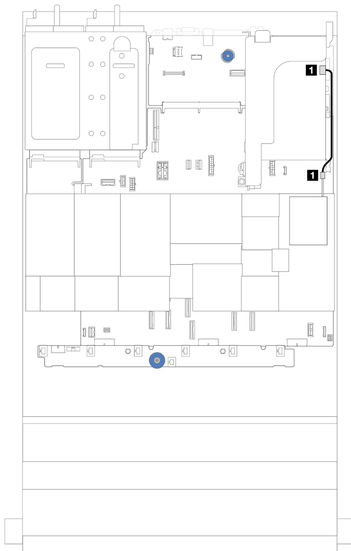
図 276. RAID フラッシュ電源モジュールのケーブル配線
