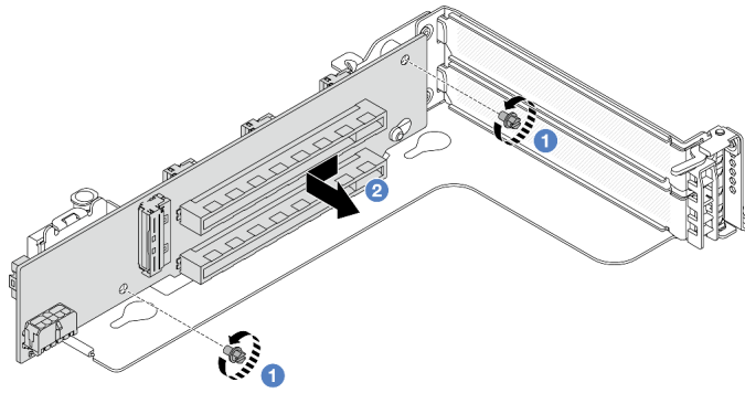
図 123. ライザー・カード 3 の取り外し
