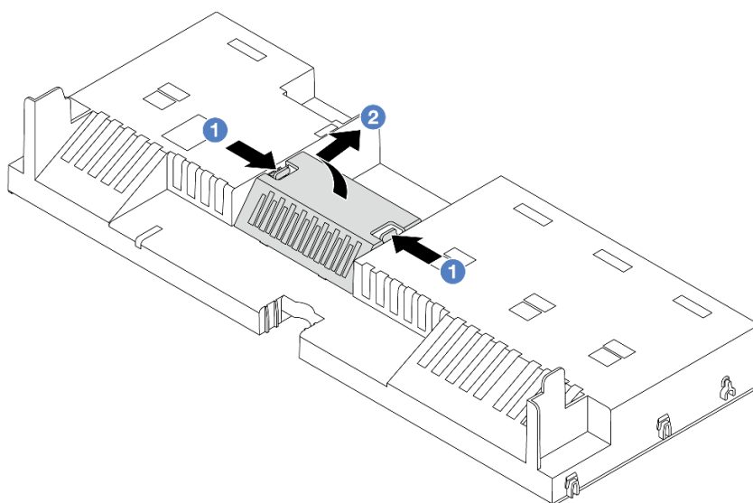
図 13. エアー・バッフル・フィルターの取り外し
