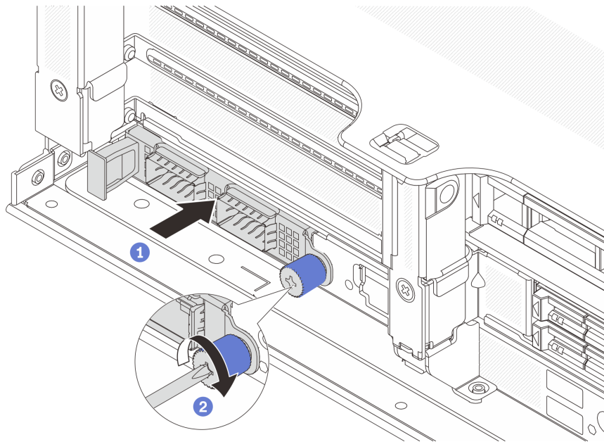
図 136. 背面 OCP モジュールの取り付け
