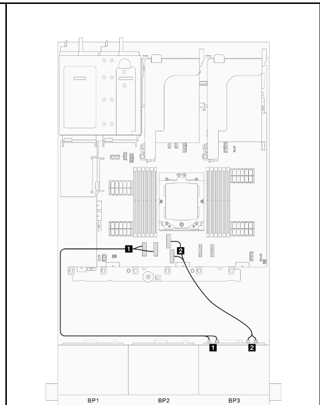
図 311. 信号ケーブルの配線、パート 2
