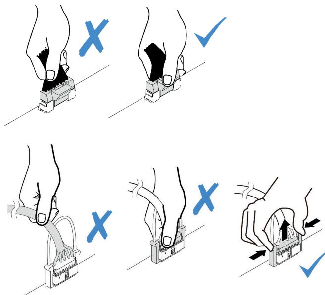
図 61. ケーブルのシステム・ボード・アセンブリーからの切り離し
