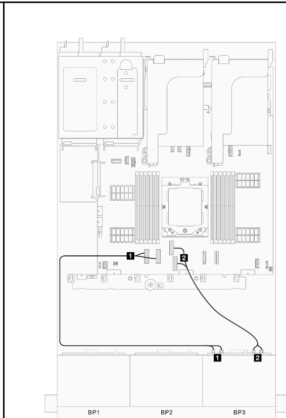
図317. 信号ケーブルの配線、パート 2
