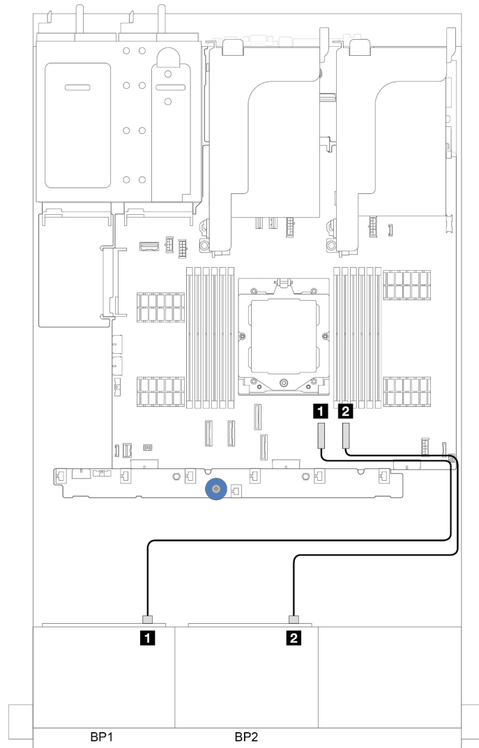
図300. オンボード SATA コネクターへの SAS/SATA ケーブル配線
