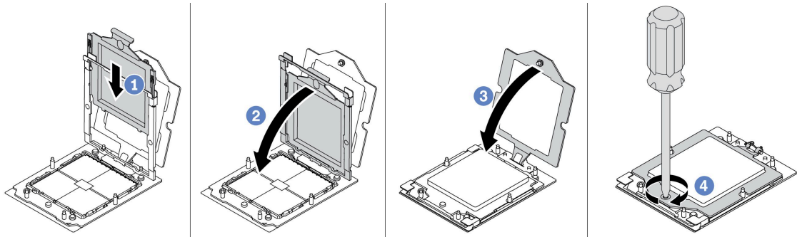
図149. プロセッサの取り付け
