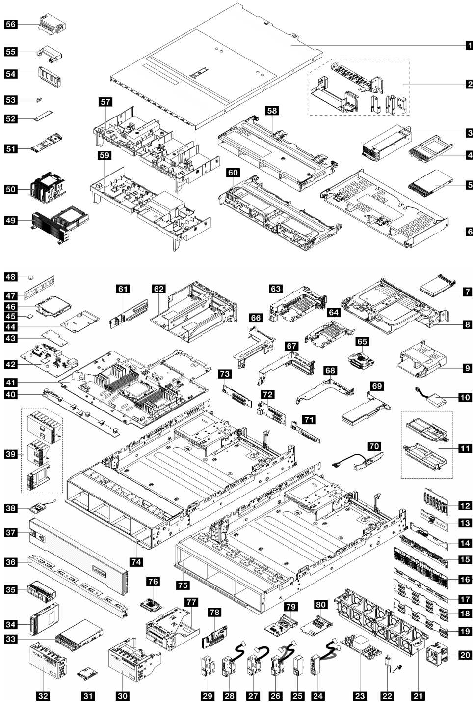
그림 19. 서버 구성 요소
