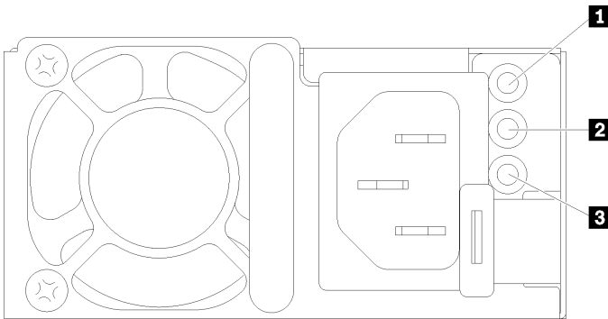
그림 16. 전원 공급 장치 LED
