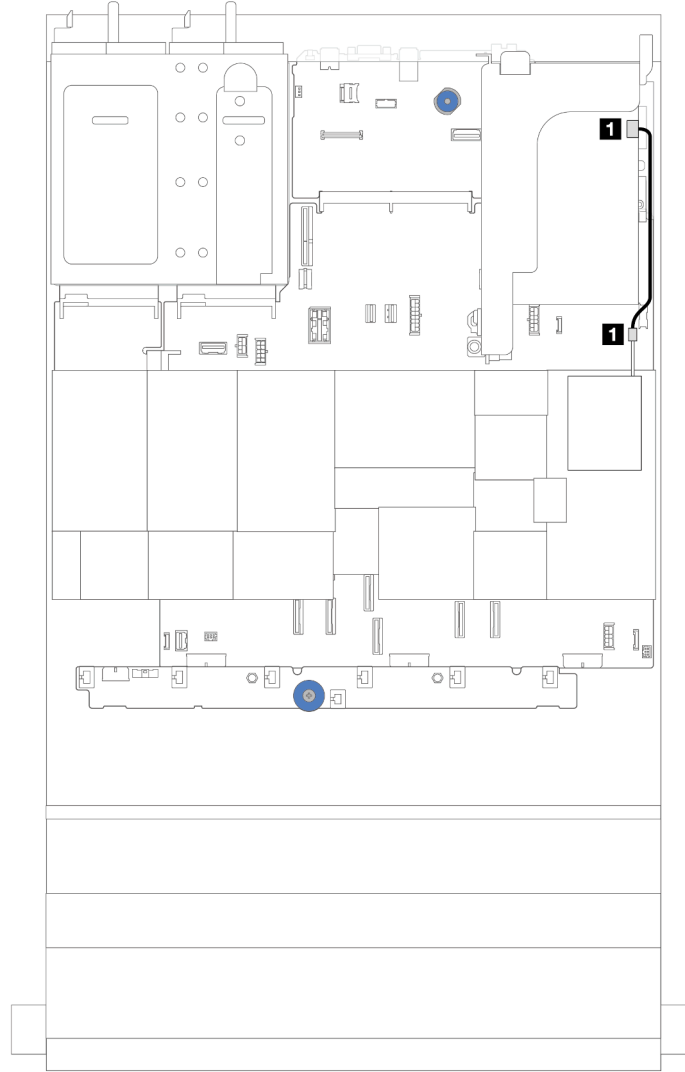
그림 291. RAID 플래시 전원 모듈의 케이블 배선
