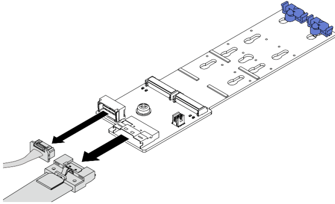
그림 109. ThinkSystem M.2 SATA/x4 NVMe 2-Bay Enablement Kit에서 M.2 케이블 분리
