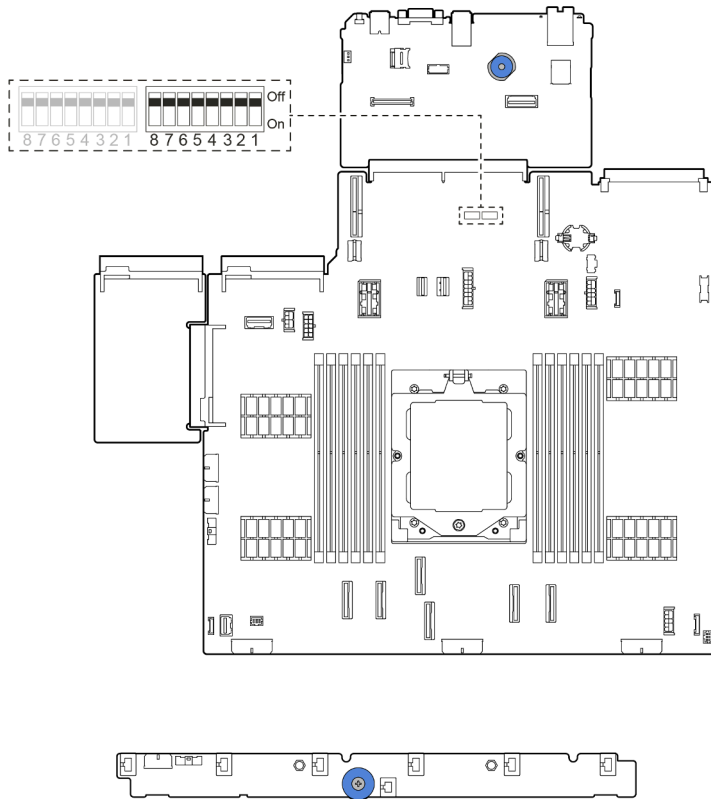
그림 12. 시스템 보드 어셈블리의 스위치 블록
