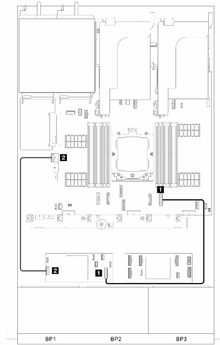
그림 345. CFF 어댑터의 신호 케이블 배선
