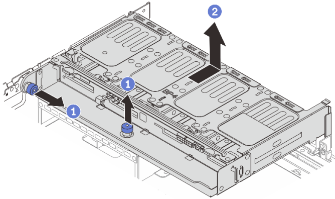
그림 217. 8 x 2.5" 뒷면 드라이브 케이스 제거
