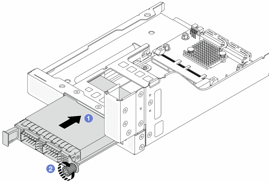
그림 40. OCP 모듈 설치
