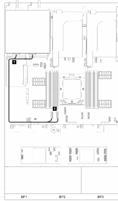
그림 347. 신호 케이블 배선 파트 2
