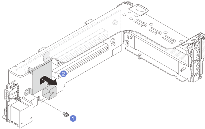
그림 204. 7mm 드라이브 케이지 고정 클립 제거
