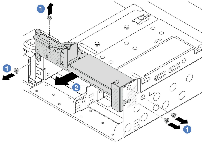
그림 197. C1 뒷면 벽 브래킷 제거(오른쪽)
