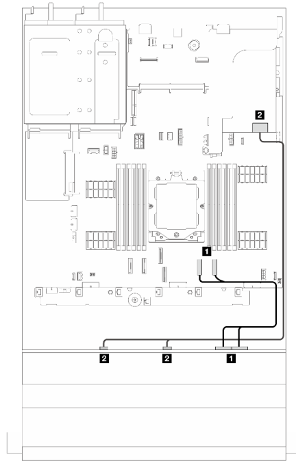
그림 383. 신호 케이블 배선(라이저 3 지원)
