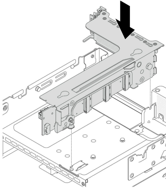
그림 147. 라이저 3 어셈블리 설치
