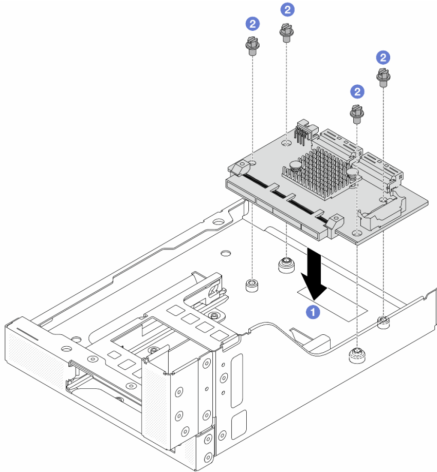
그림 39. 앞면 OCP 인터포저 카드 설치
