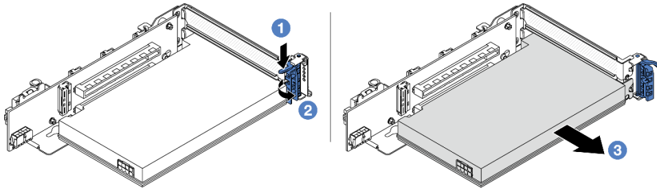
그림 135. 라이저 3 어셈블리에서 PCIe 어댑터 제거
