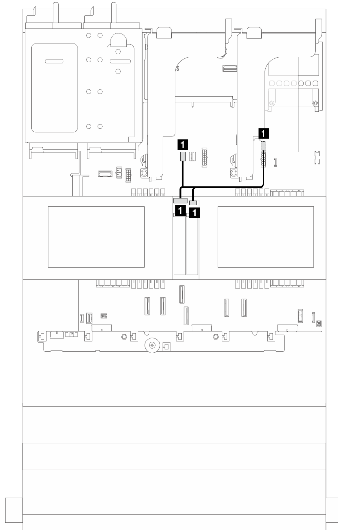
그림 285. M.2 드라이브 백플레인의 케이블 배선
