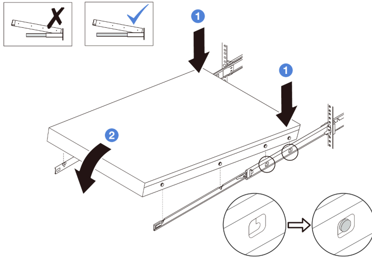
그림 23. 레일에 서버 설치
