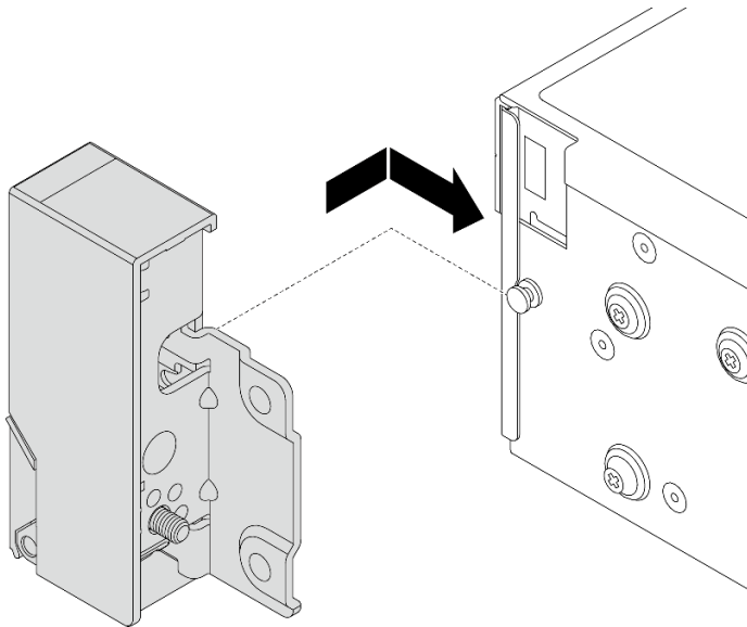
그림 172. 랙 래치 설치
