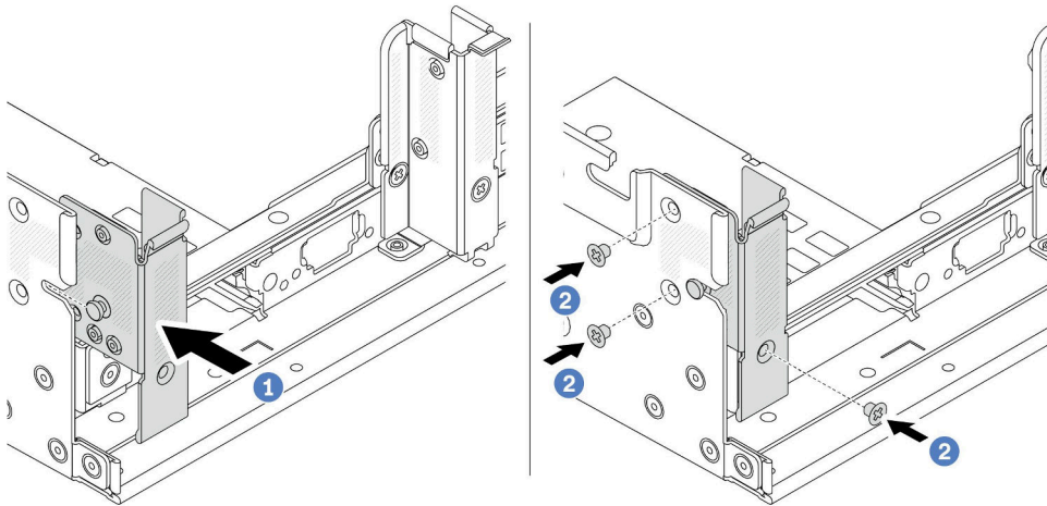
그림 198. A1 뒷면 벽 브래킷 설치(왼쪽)
