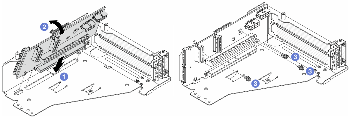
그림 41. 라이저 카드 설치
