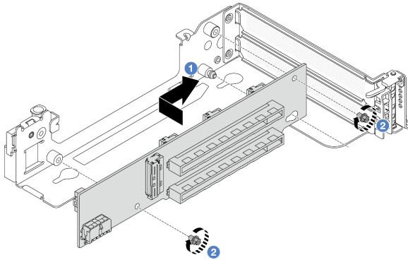
그림 141. 라이저 카드 3 설치
