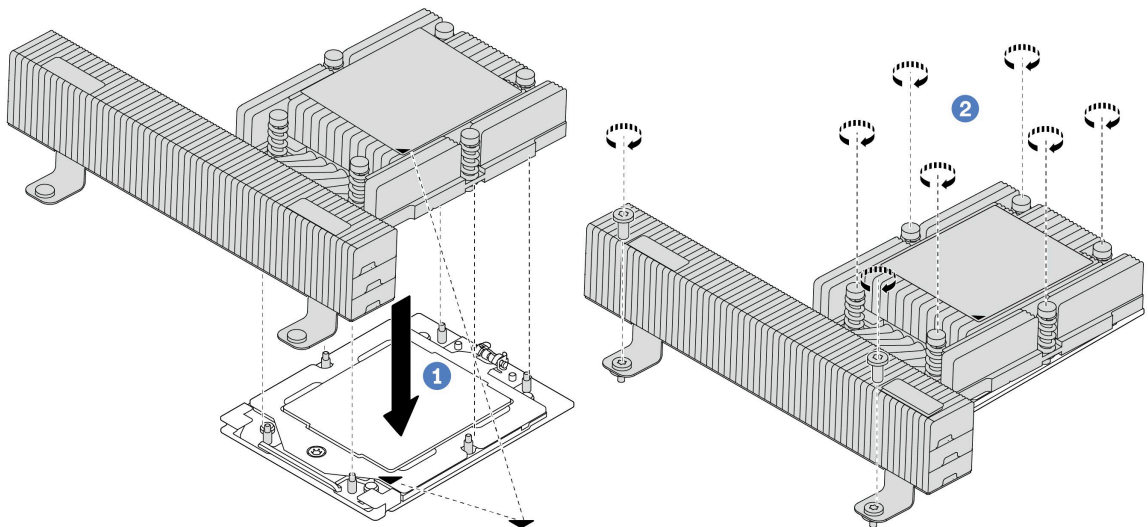
그림 167. 성능 방열판 설치
