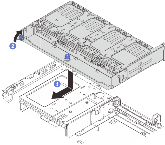
그림 220. 8 x 2.5" 드라이브 후면 케이지 설치
