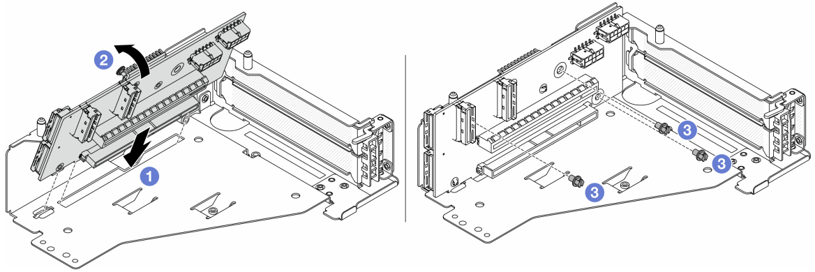
그림 61. 라이저 카드 설치
