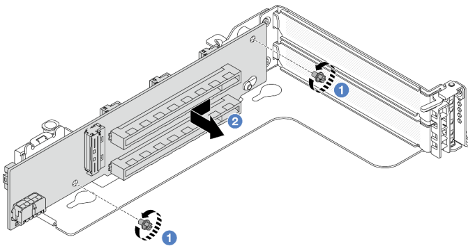
그림 138. 라이저 카드 3 제거
