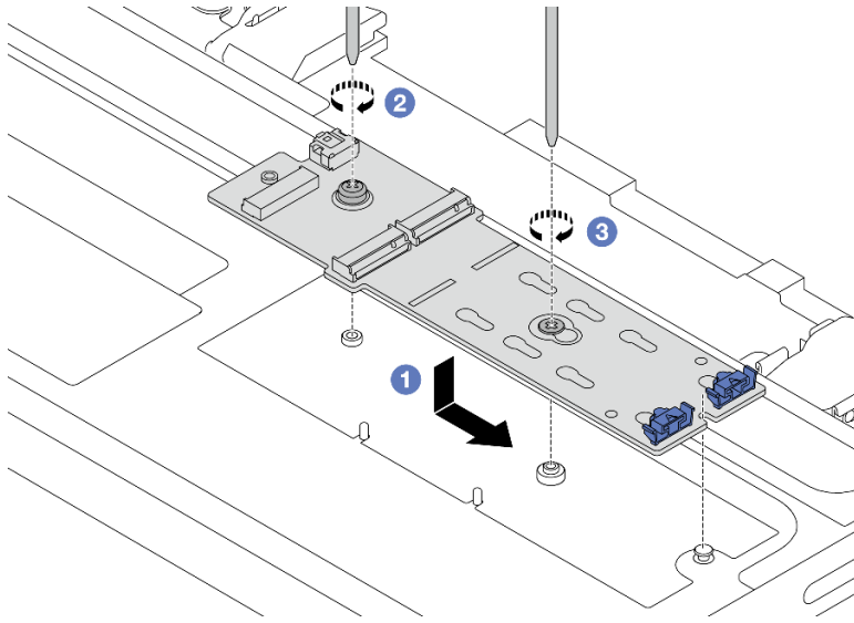
그림 114. 중간 드라이브 케이스에 M.2 백플레인 설치
