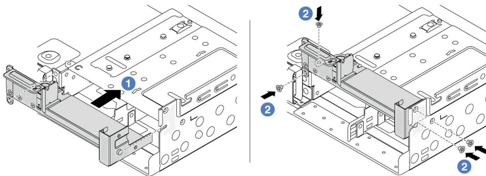
그림 200. C1 뒷면 벽 브래킷 설치(오른쪽)
