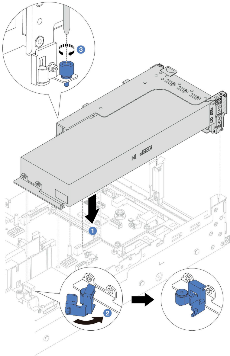
그림 90. GPU 어댑터로 라이저 1 어셈블리 설치
