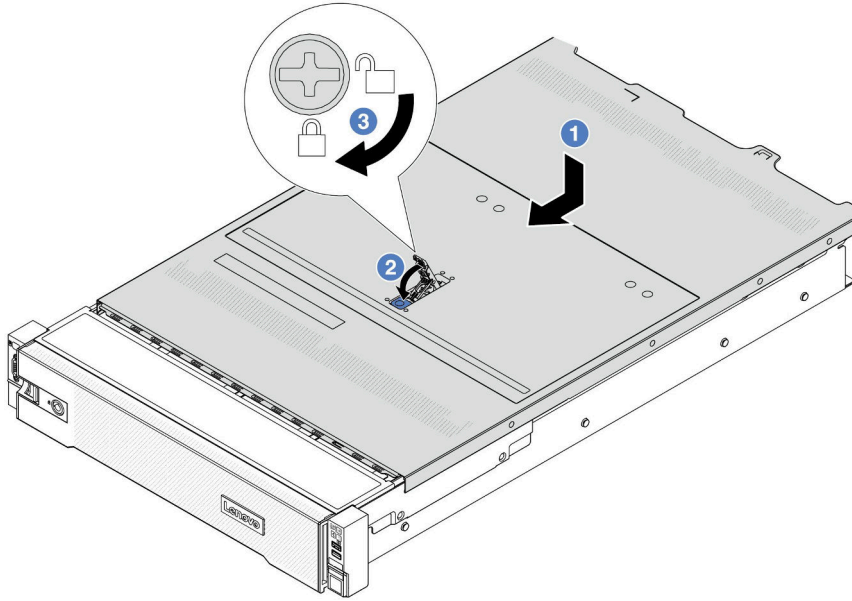
그림 254. 윗면 덮개 설치
