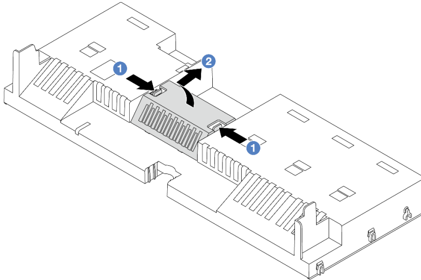
그림 28. 공기 조절 장치 필터 제거
