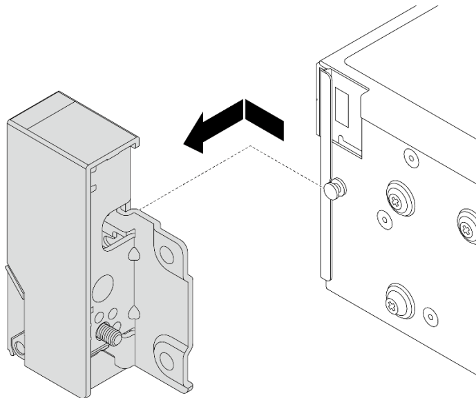
그림 171. 래치 제거
