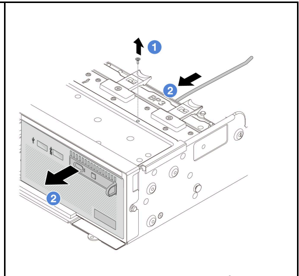
그림 78. 내장형 진단 패널 포함 앞면 I/O 모듈
