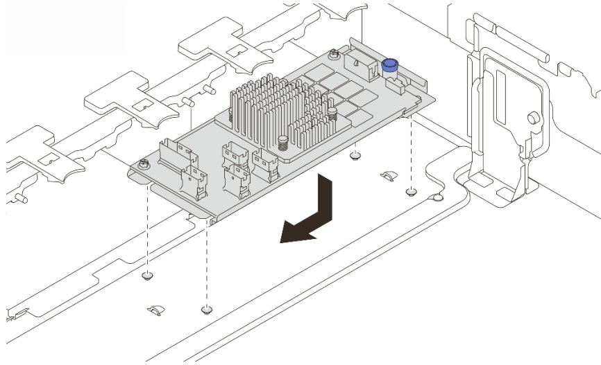
그림 100. 내부 CFF 어댑터 설치
