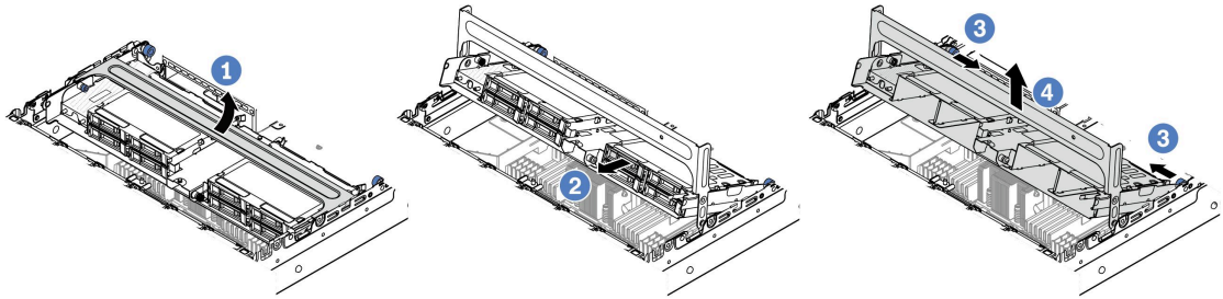
그림 124. 중간 드라이브 케이스 제거
