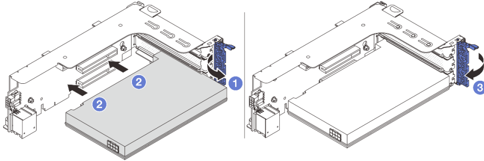
그림 143. 라이저 1 또는 2 어셈블리에 PCIe 어댑터 설치
