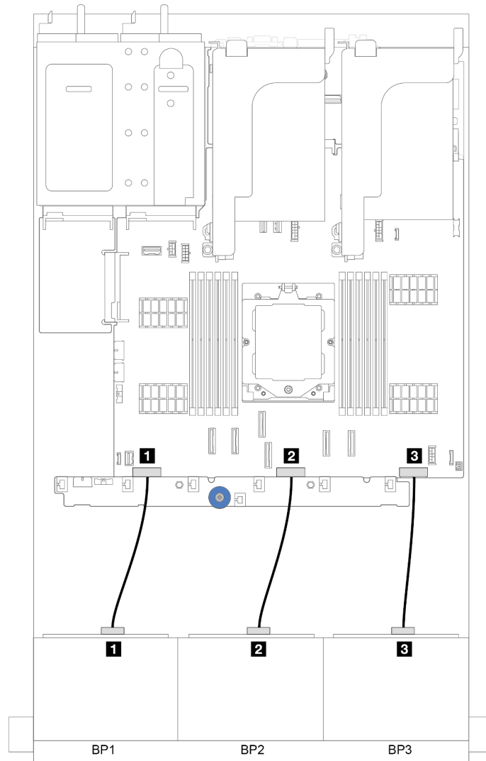
그림 301. 8 x 2.5" 앞면 드라이브 백플레인의 전원 케이블 연결
