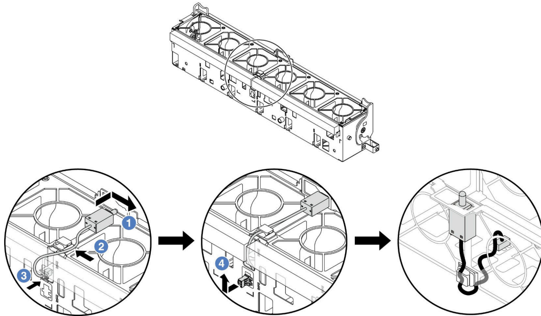
그림 103. 침입 스위치 설치
