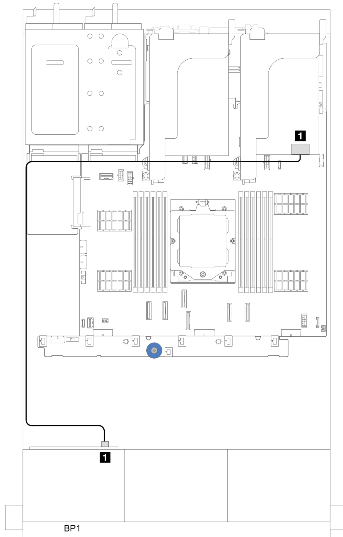
그림 308. 8i/16i RAID/HBA 어댑터에 대한 SAS/SATA 케이블 배선
