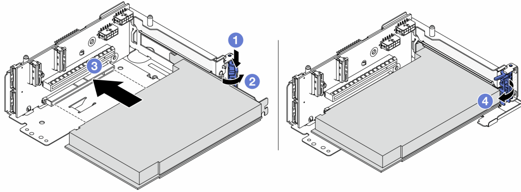
그림 42. 라이저 5 케이스에 PCIe 어댑터 설치
