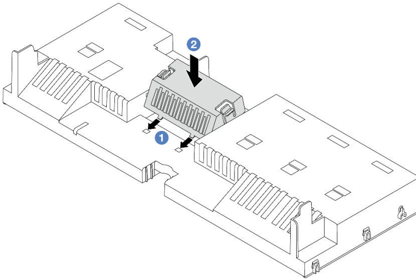
그림 29. 공기 조절 장치 필터 설치
