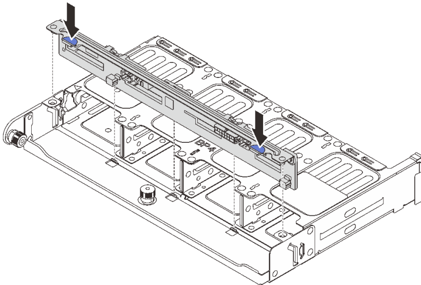
그림 219. 8 x 2.5" 뒷면 드라이브 백플레인 설치
