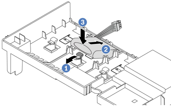
그림 188. 공기 조절 장치에 RAID 플래시 전원 모듈 설치
