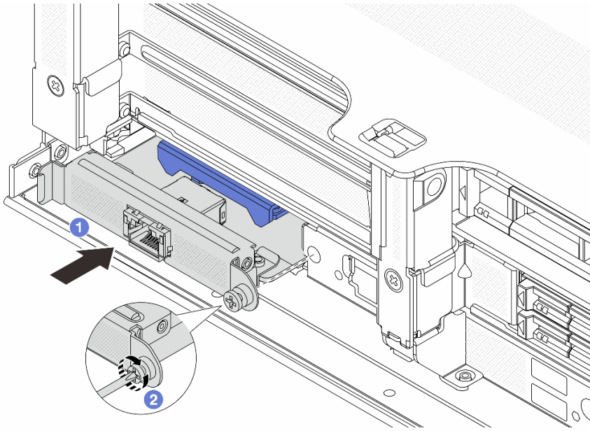
그림 119. 관리 NIC 어댑터 설치
