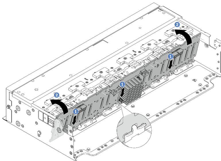
그림 71. 24베이 확장기 백플레인 설치
