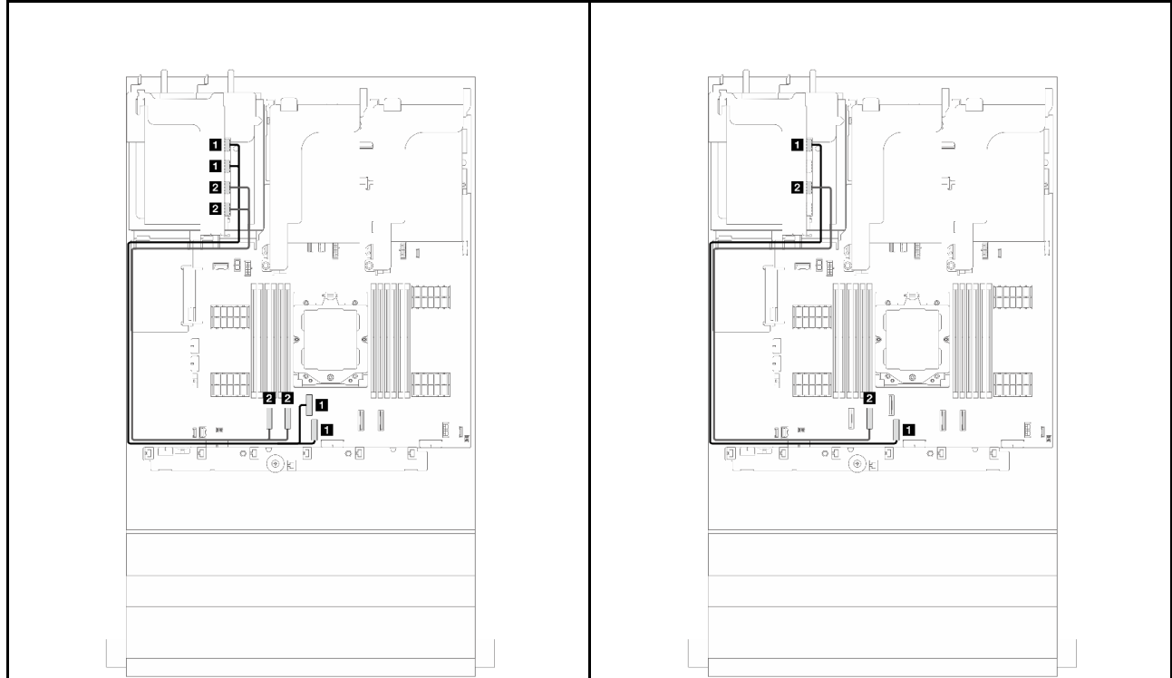
그림 293. 라이저 3(x16/x16 Gen 5) 신호 케이블 배선
