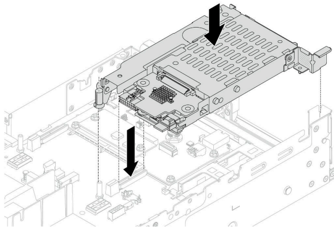
그림 212. 7mm SSD 라이저 케이스 설치
