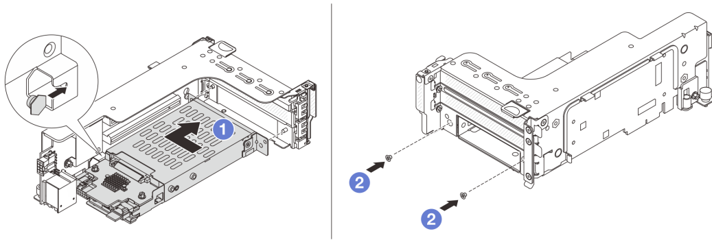
그림 210. 라이저 어셈블리에 7mm 드라이브 케이지 설치
