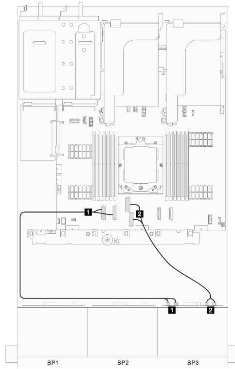
그림 332. 신호 케이블 배선 파트 2
