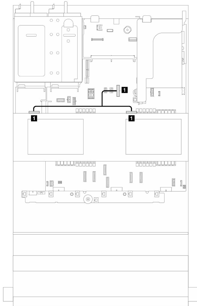
그림 303. 중간 드라이브 백플레인의 전원 케이블 연결
