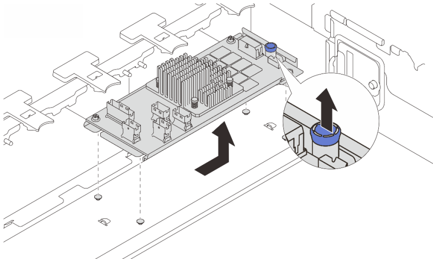
그림 99. 내부 CFF 어댑터 제거
