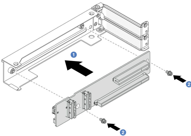
그림 142. 4LP 라이저 3/4 케이스에 라이저 카드 설치
