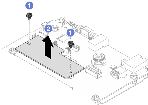
그림 236. 펌웨어 및 RoT 보안 모듈 제거
