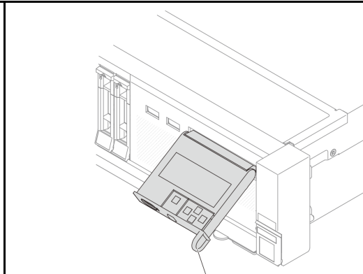
1 LCD 디스플레이가 있는 내장형 진단 패널
