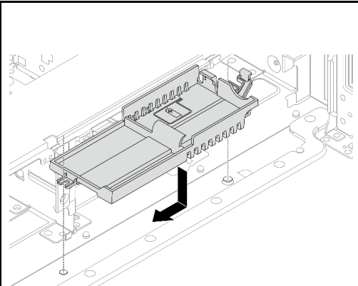
그림 184. Supercap Holder 설치
