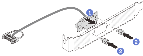
그림 250. 직렬 포트 모듈 조립
