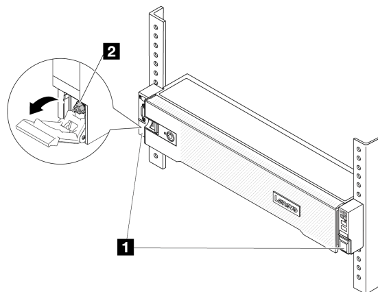
그림 26. 랙의 앞면에 서버 고정
