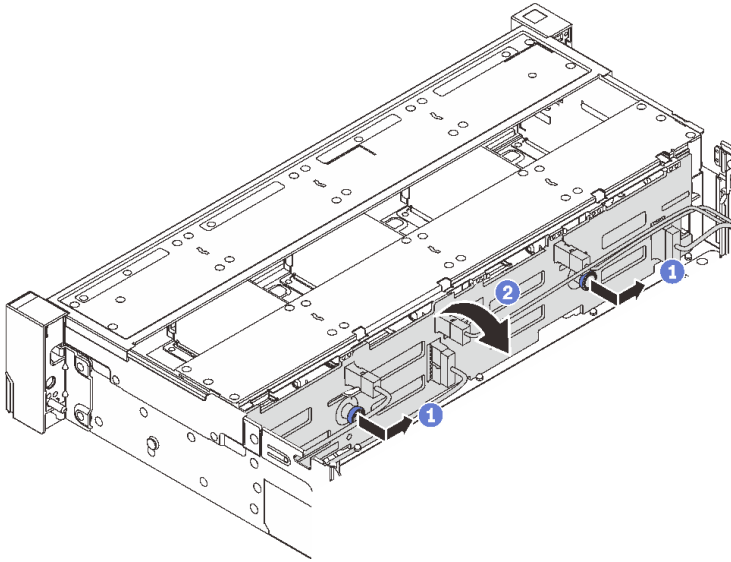
그림 72. 3.5" 드라이브 백플레인 제거
