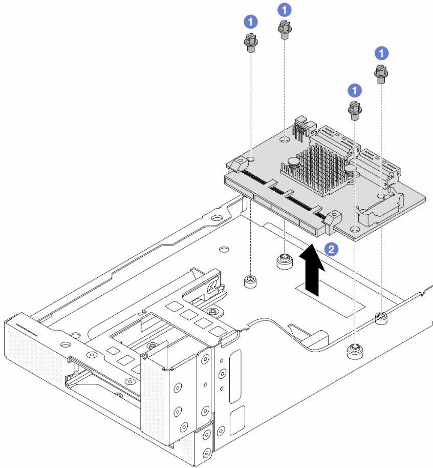
그림 38. 앞면 OCP 인터포저 카드 제거
