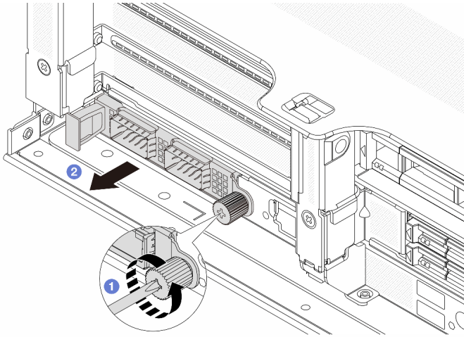
그림 150. 뒷면 OCP 모듈 제거
