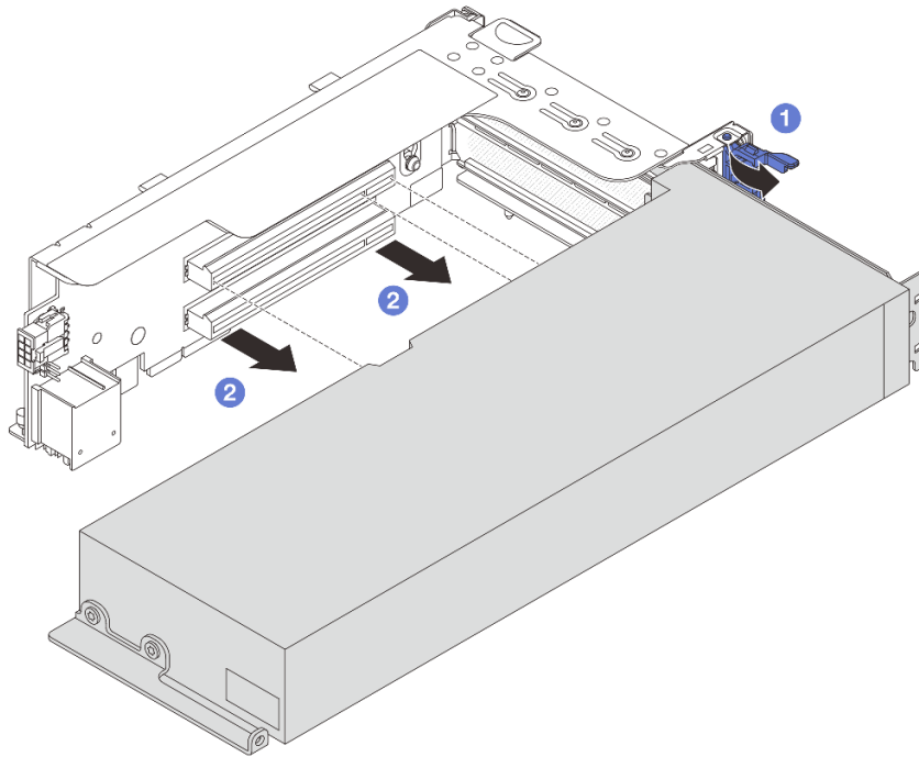
그림 87. GPU 어댑터 제거
