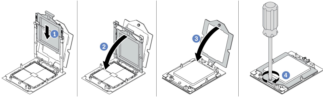
그림 164. 프로세서 설치
