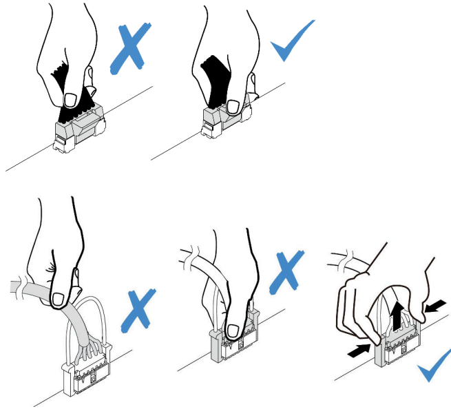
그림 98. 시스템 보드 어셈블리에서 케이블 분리
