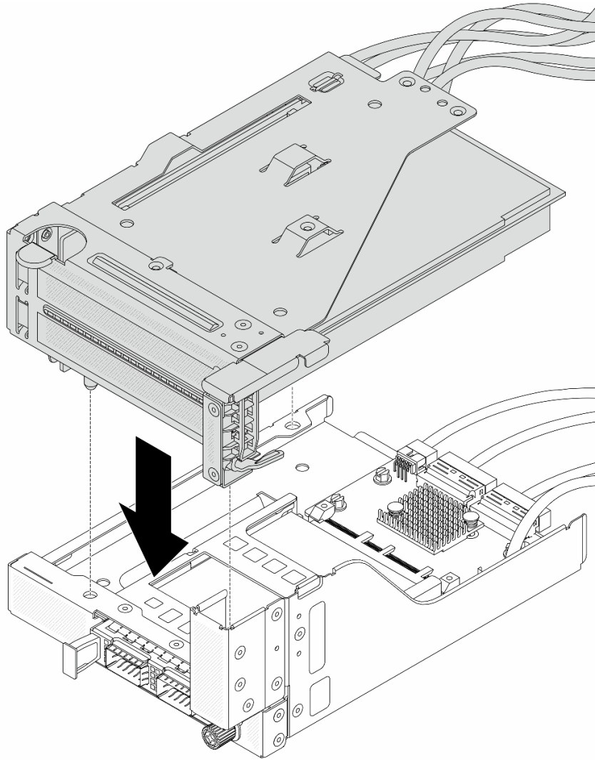
그림 53. 앞면 OCP 어셈블리에 레이저 5 어셈블리 설치
