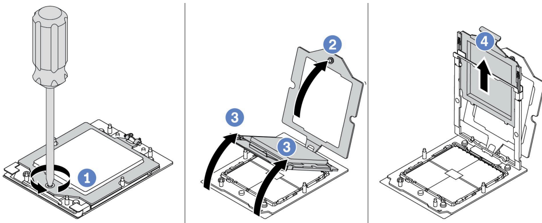
그림 163. 프로세서 제거
