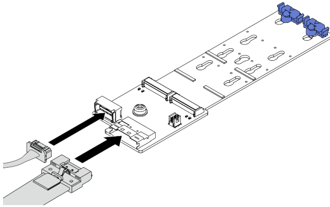
그림 116. ThinkSystem M.2 SATA/x4 NVMe 2-Bay Enablement Kit에 M.2 케이블 연결
