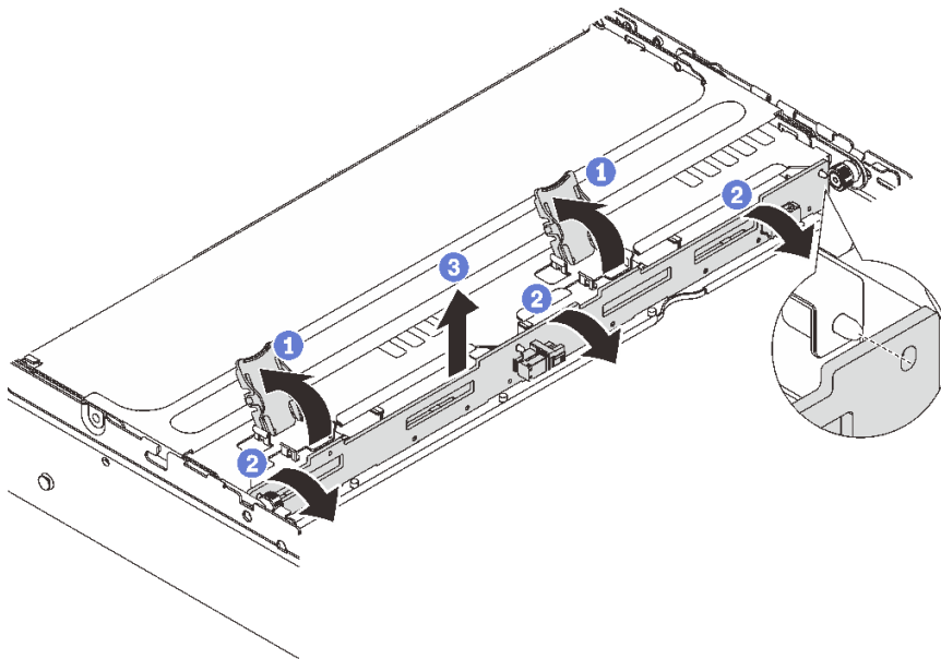
그림 126. 중간 3.5" 드라이브 백플레인 제거
