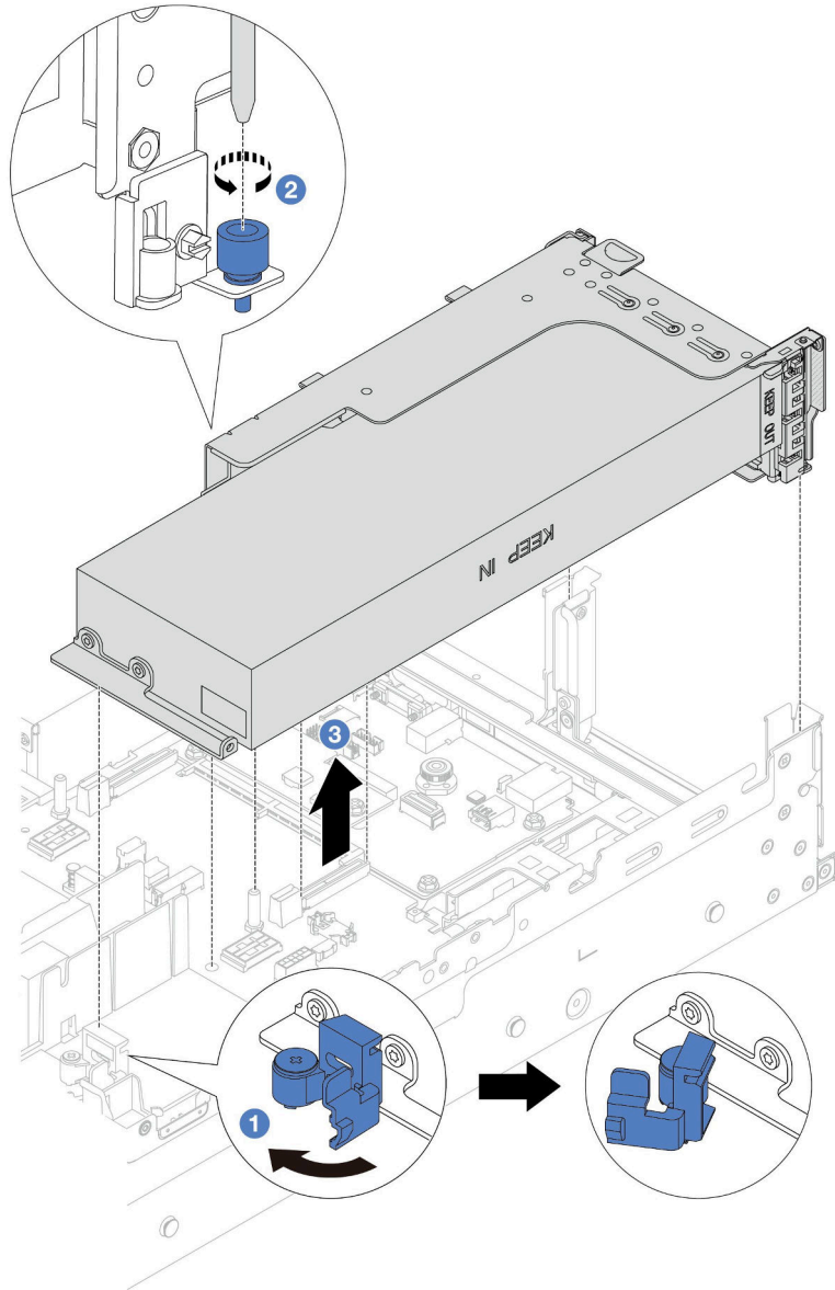
그림 85. GPU 어댑터로 라이저 1 어셈블리 제거
