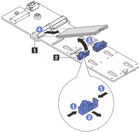
그림 104. M.2 드라이브 제거
