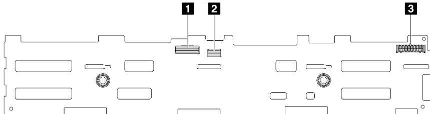
그림 261. 12 x 3.5" SAS/SATA 확장기 백플레인의 커넥터
