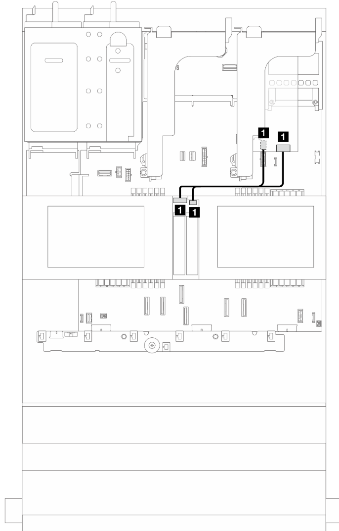
그림 282. M.2 드라이브 백플레인의 RAID 케이블 배선
