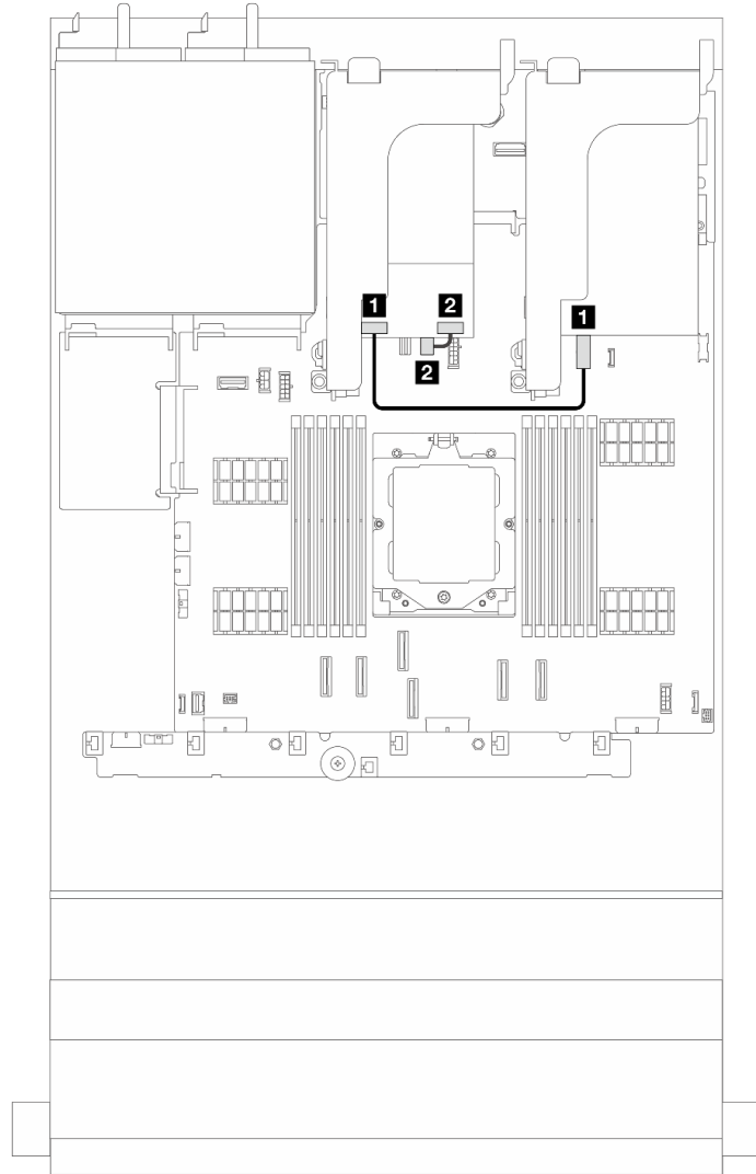
그림 271. 7mm 드라이브 백플레인의 NVMe 케이블 배선
