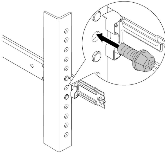
그림 25. 랙의 뒷면에 서버 고정
