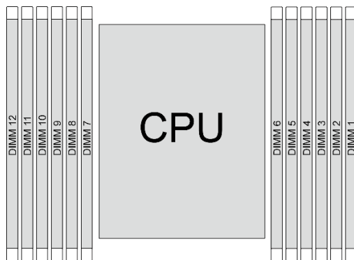
그림 16. 메모리 모듈 및 프로세서 레이아웃
