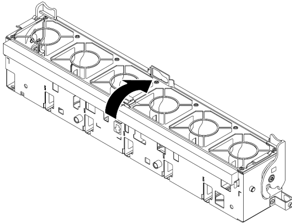
그림 101. 팬 케이스 회전
