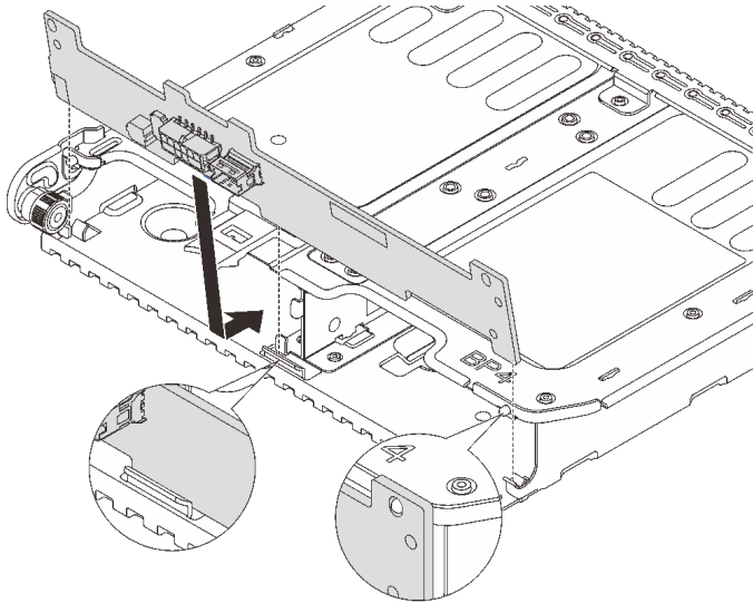
그림 223. 2 x 3.5" 뒷면 드라이브 백플레인 설치
