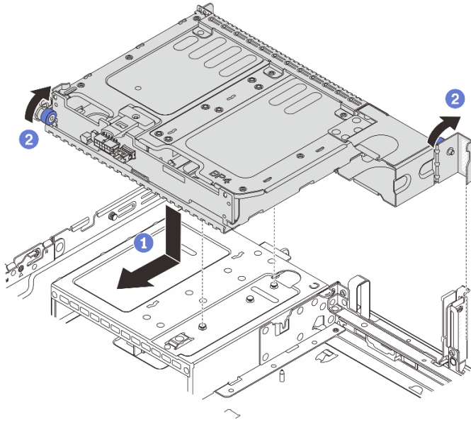
그림 224. 2 x 3.5" 드라이브 후면 케이지 설치
