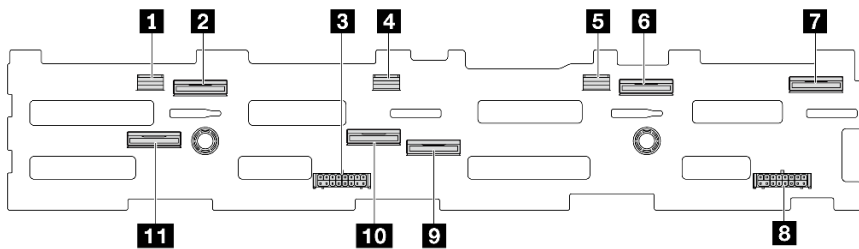
그림 262. 12 x 3.5" AnyBay 백플레인 커넥터
