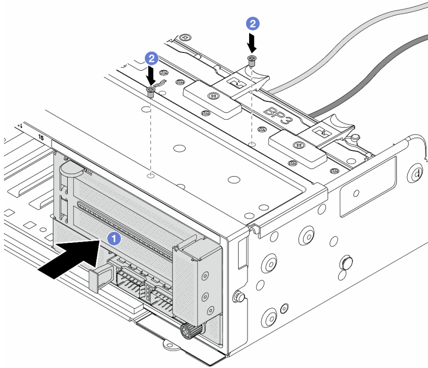
그림 64. 앞면 어댑터 어셈블리 설치
