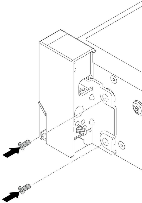
그림 173. 나사 설치
