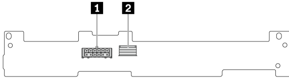
그림 266. 2 x 3.5" SAS/SATA 백플레인 커넥터
