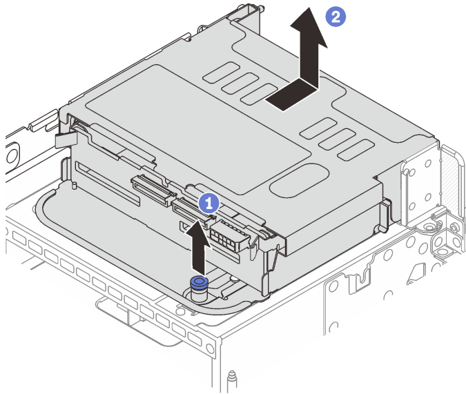
그림 213. 4 x 2.5" 뒷면 드라이브 케이지 제거
