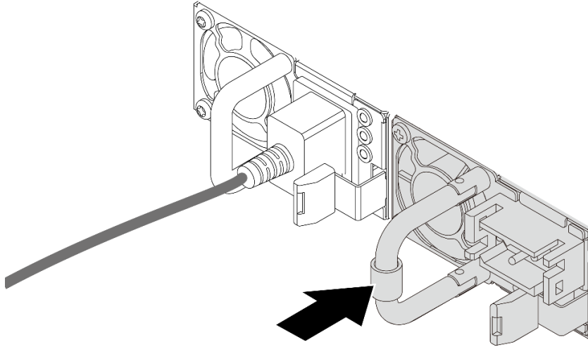
그림 159. 전원 공급 장치 설치
