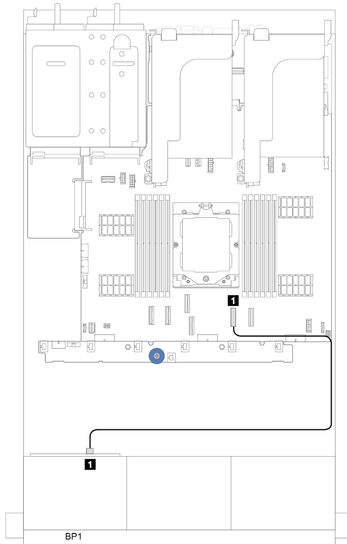
그림 305. 온보드 SATA 커넥터에 대한 SAS/SATA 케이블 배선
