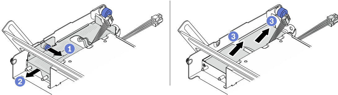
그림 191. 중간 드라이브 케이지에서 RAID 플래시 전원 모듈 제거
