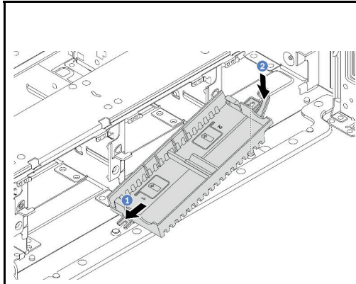
그림 183. Supercap Holder 설치
