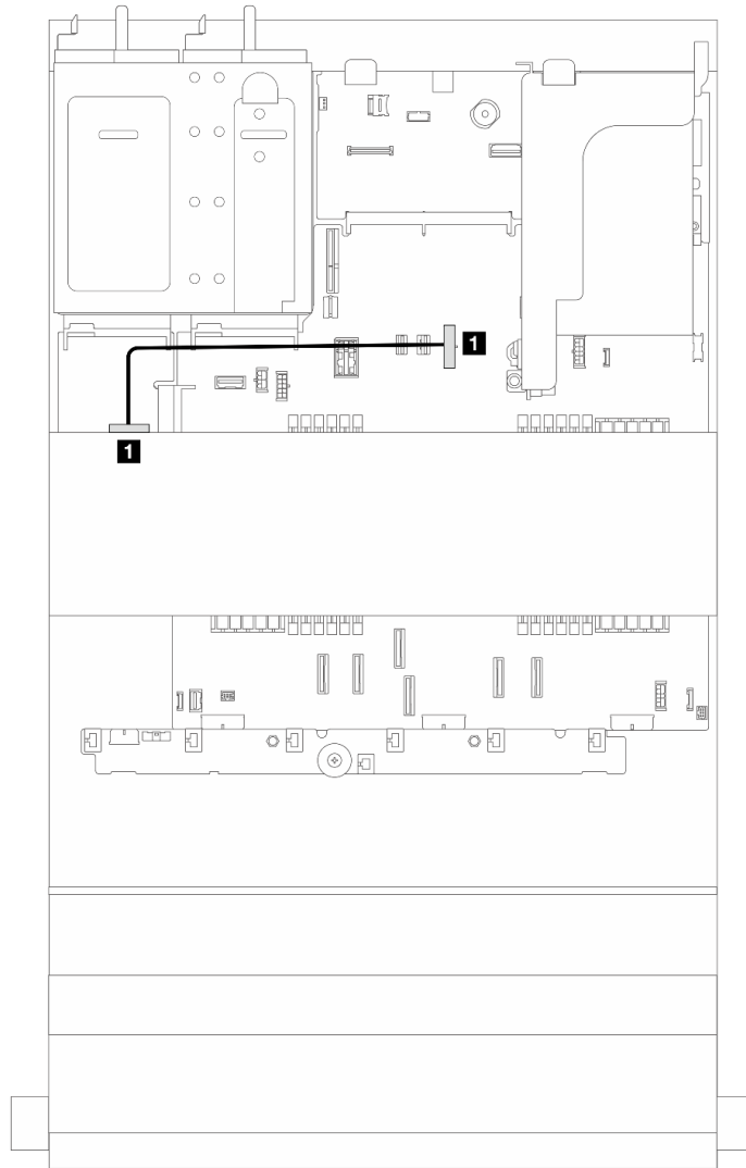
그림 377. 4 x 2.5" 또는 4 x 3.5" 중간 드라이브 백플레인 1개의 전원 케이블 배선
