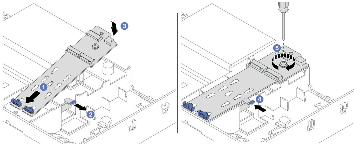
그림 113. 공기 조절 장치에 M.2 백플레인 설치
