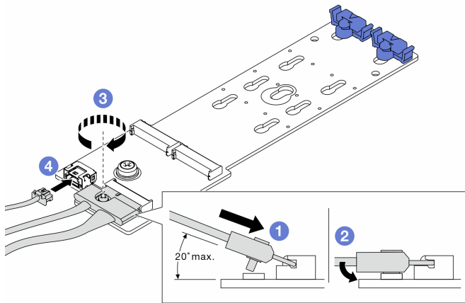
그림 115. ThinkSystem M.2 SATA/NVMe 2-Bay Enablement Kit 또는 ThinkSystem M.2 NVMe 2-Bay RAID Enablement Kit에 M.2 케이블 연결
