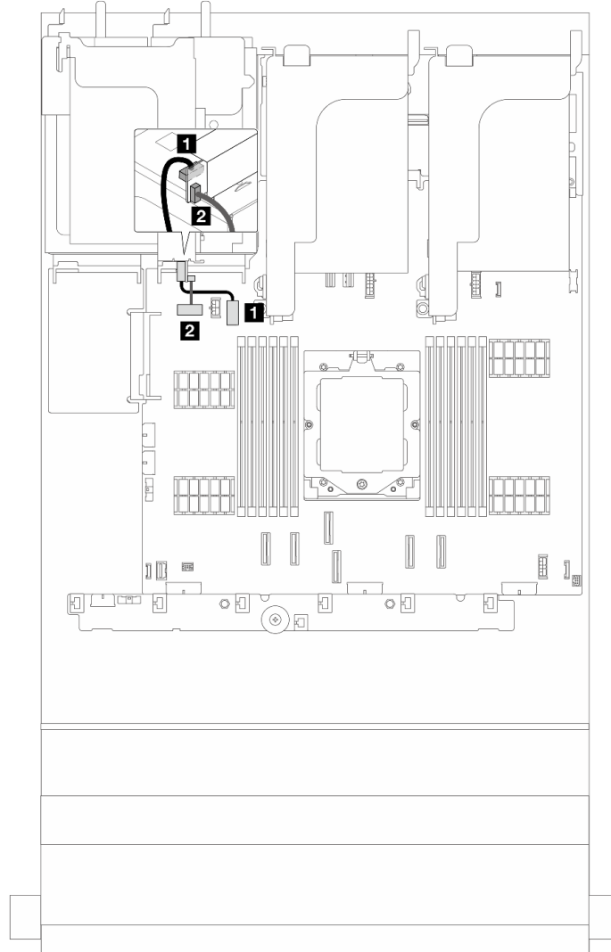
그림 292. 라이저 3 전원 및 사이드밴드 연결(Gen4/Gen5)
