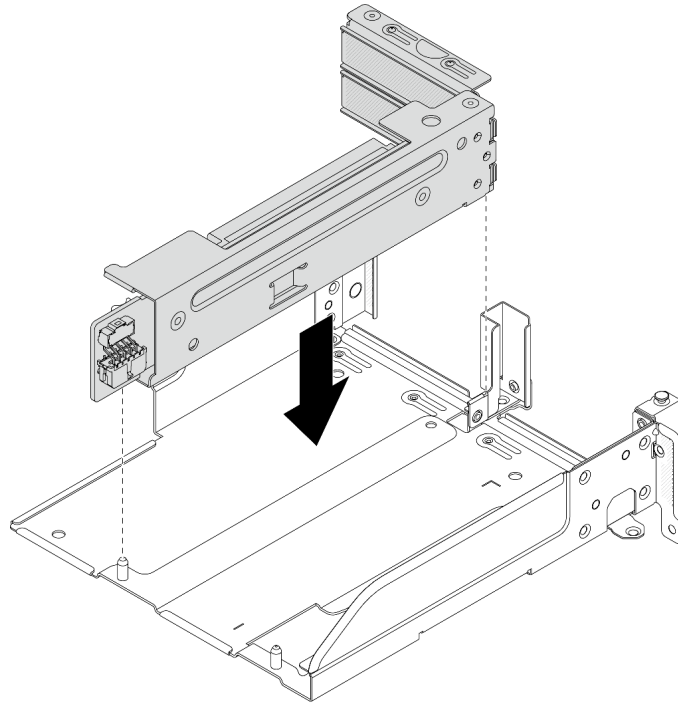
그림 149. 라이저 3/4 어셈블리 설치
