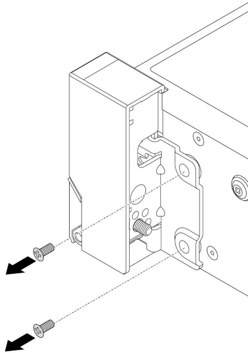
그림 170. 나사 제거
