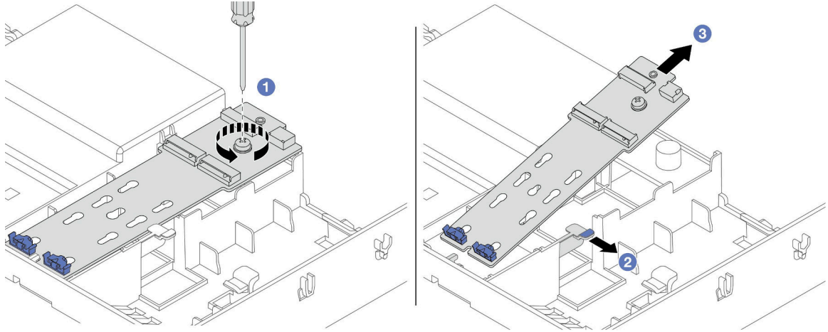
그림 111. 공기 조절 장치에서 M.2 백플레인 제거
