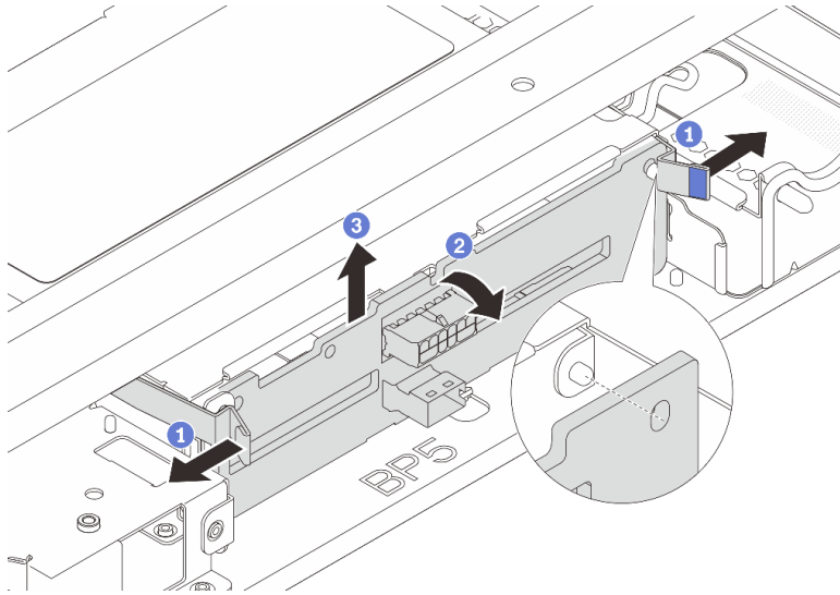
그림 125. 중간 2.5" 드라이브 백플레인 제거
