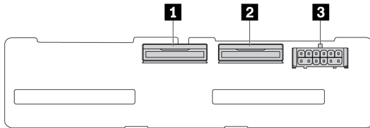
그림 264. 4 x 2.5" NVMe 백플레인 커넥터
