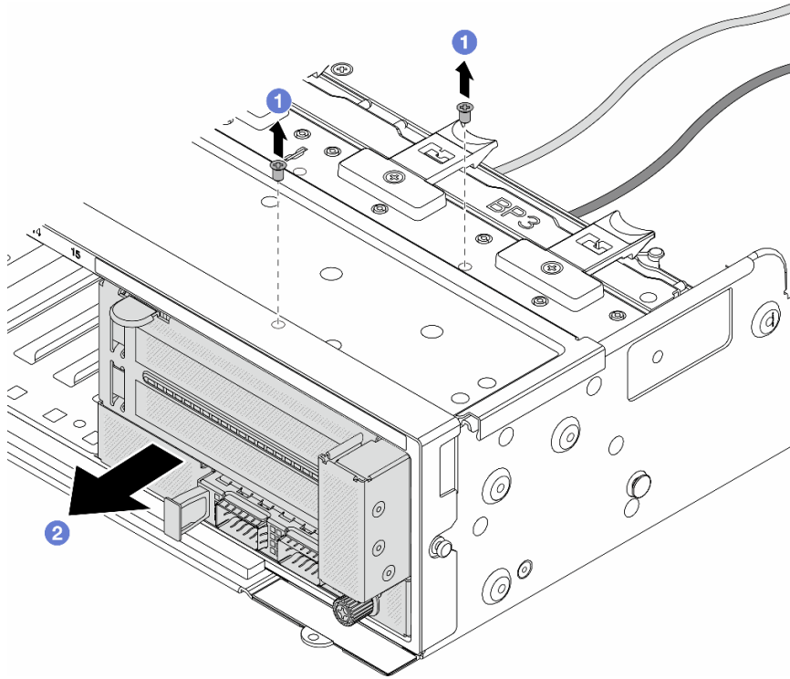
그림 33. 앞면 어댑터 어셈블리 제거
