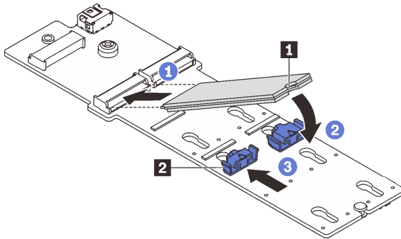
그림 107. M.2 드라이브 설치
