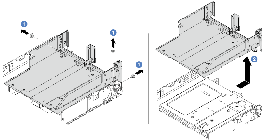
그림 133. 라이저 케이스 트레이 제거
