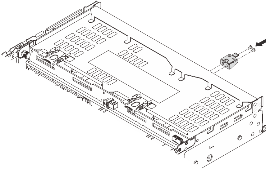
그림 229. 상단 덮개 지원 브라켓 설치
