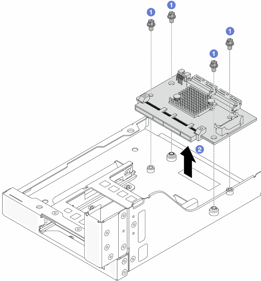
그림 50. 앞면 OCP 인터포저 카드 제거
