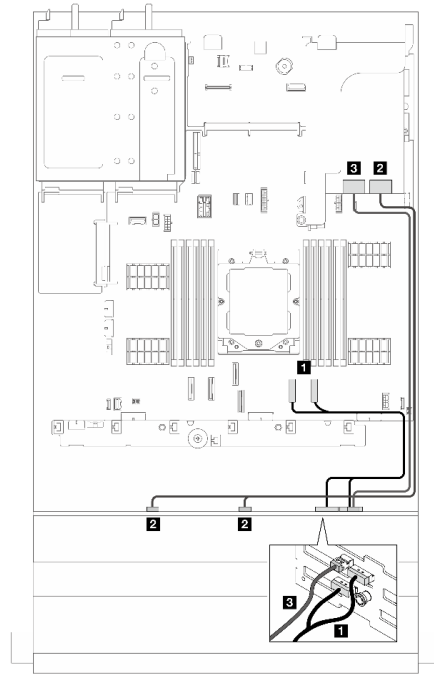
그림 385. 신호 케이블 배선(라이저 3 지원)
