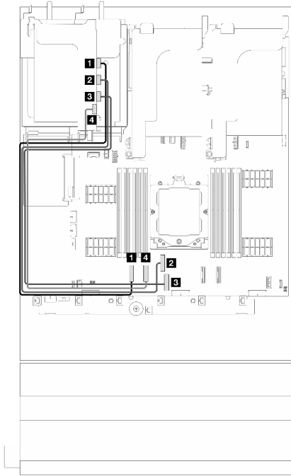
그림 295. 라이저 3(x16/x16 Gen 4) 신호 케이블 배선
