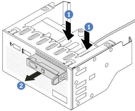
그림 79. 내장형 진단 패널 제거
