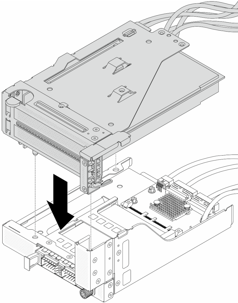
그림 43. 앞면 OCP 어셈블리에 라이저 5 어셈블리 설치
