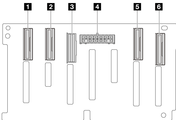
그림 257. 8 x 2.5" AnyBay 백플레인 커넥터
