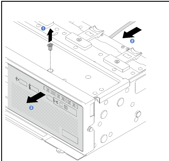
그림 77. 앞면 오퍼레이터 패널 포함 앞면 I/O 모듈
