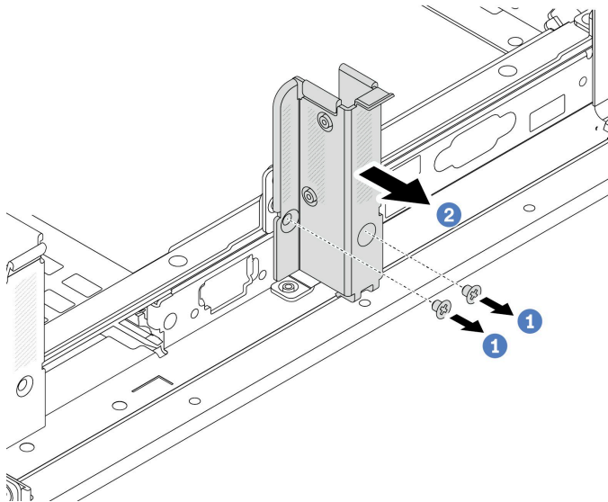
그림 196. B1 뒷면 벽 브래킷 제거(중간)
