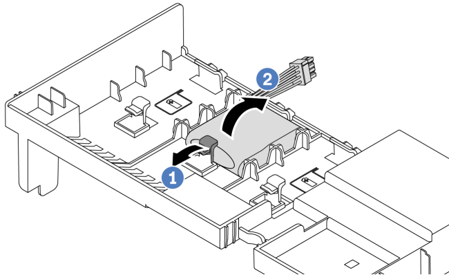
그림 187. 공기 조절 장치에서 RAID 플래시 전원 모듈 제거
