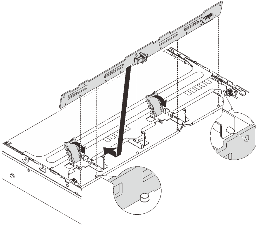
그림 128. 중간 3.5" 드라이브 백플레인 설치
