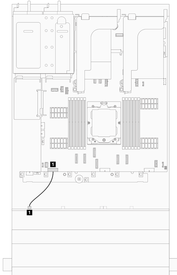
그림 374. 12 x 3.5" SAS/SATA 확장기 앞면 드라이브 백플레인의 전원 케이블 배선
