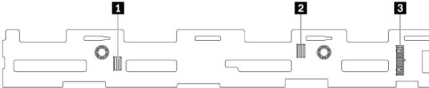
그림 259. 8 x 3.5" SAS/SATA 백플레인 커넥터
