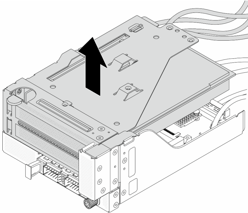
그림 34. 라이저 5 어셈블리 들어 올리기
