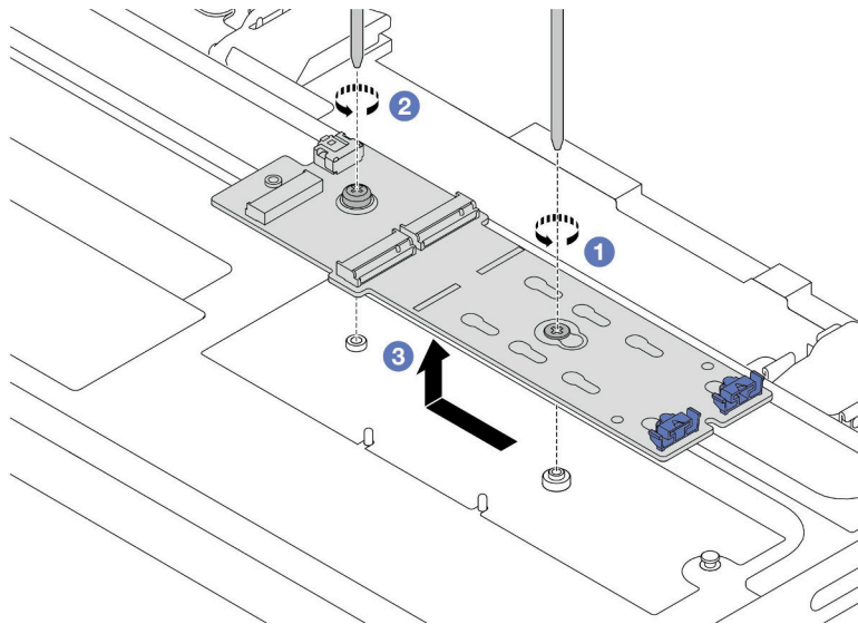
그림 112. 중간 드라이브 케이지에서 M.2 백플레인 제거
