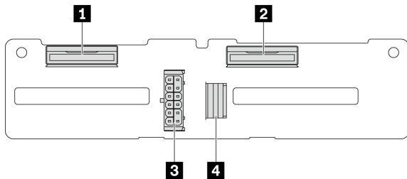
그림 268. 4 x 2.5" AnyBay 백플레인 커넥터
