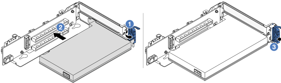
그림 144. 라이저 3 어셈블리에 PCIe 어댑터 설치
