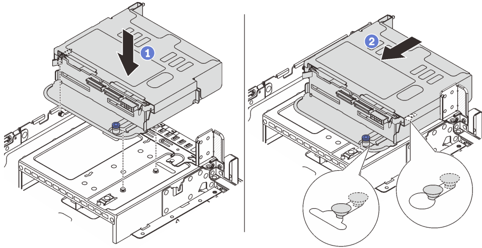
그림 216. 4 x 2.5" 드라이브 후면 케이스 설치
