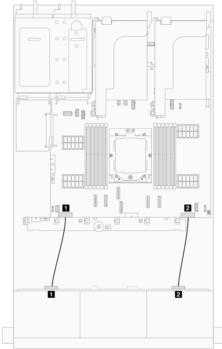
그림 302. 24 x 2.5" SAS/SATA 확장기 드라이브 백플레인의 전원 케이블 연결
