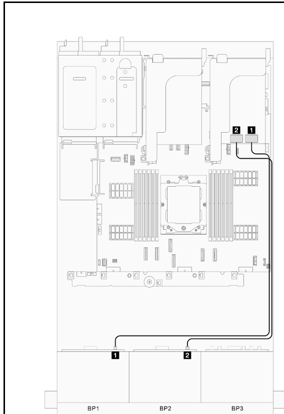
그림 329. 신호 케이블 배선 파트 1
