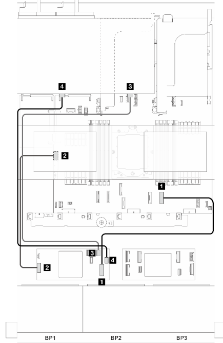
그림 360. 신호 케이블 배선 파트 2
