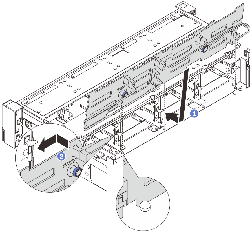
그림 73. 3.5" 드라이브 백플레인 설치
