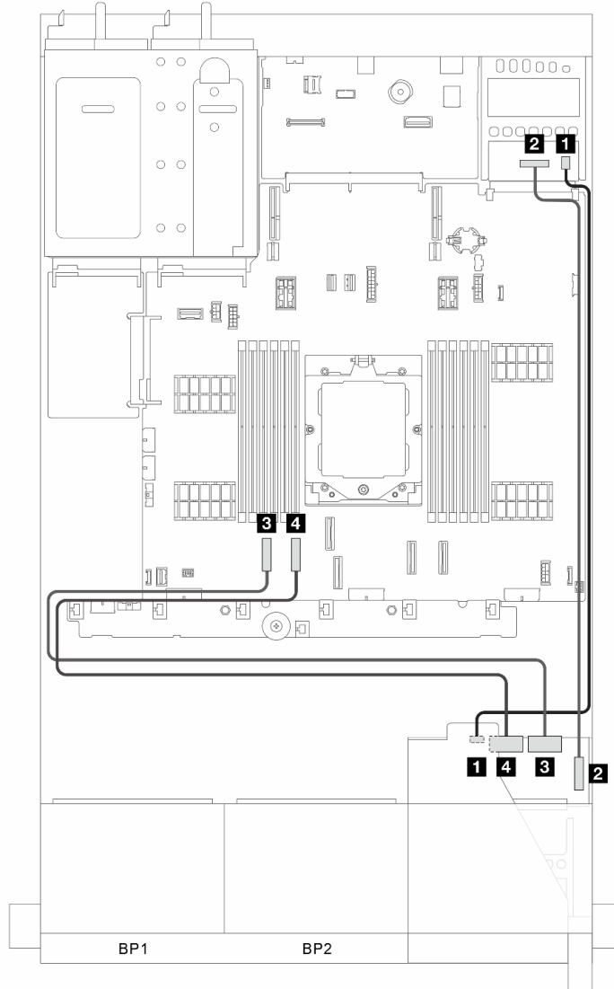
그림 290. 앞면 및 뒷면 OCP 인터포저 카드의 케이블 배선
