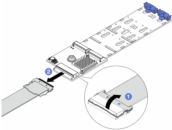
그림 110. ThinkSystem M.2 RAID B540i-2i SATA/NVMe Enablement Kit에서 M.2 케이블 분리
