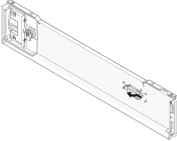
그림 232. 키 제거
