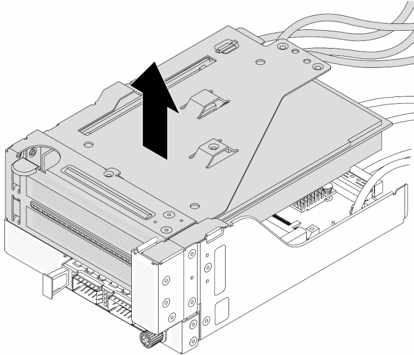
그림 48. 라이저 5 어셈블리 들어 올리기
