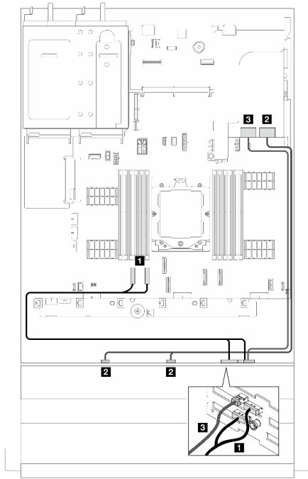
그림 384. 신호 케이블 배선
