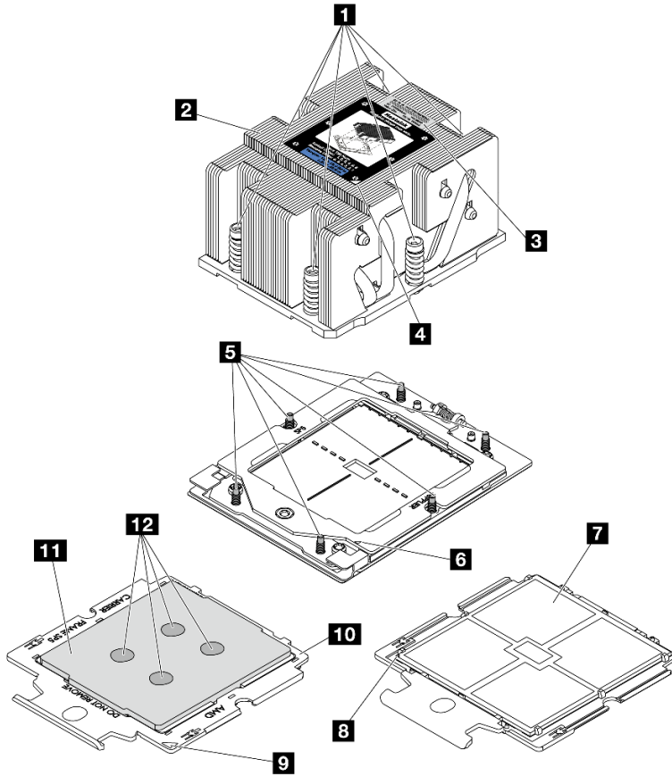
그림 160. 프로세서 및 방열판 구성 요소
