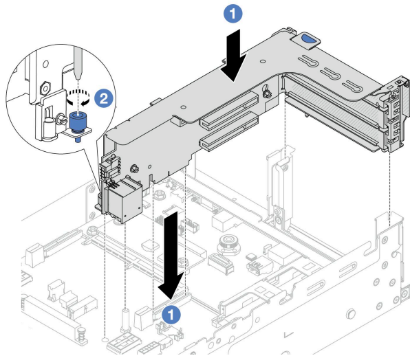
그림 146. 라이저 1 어셈블리 설치
