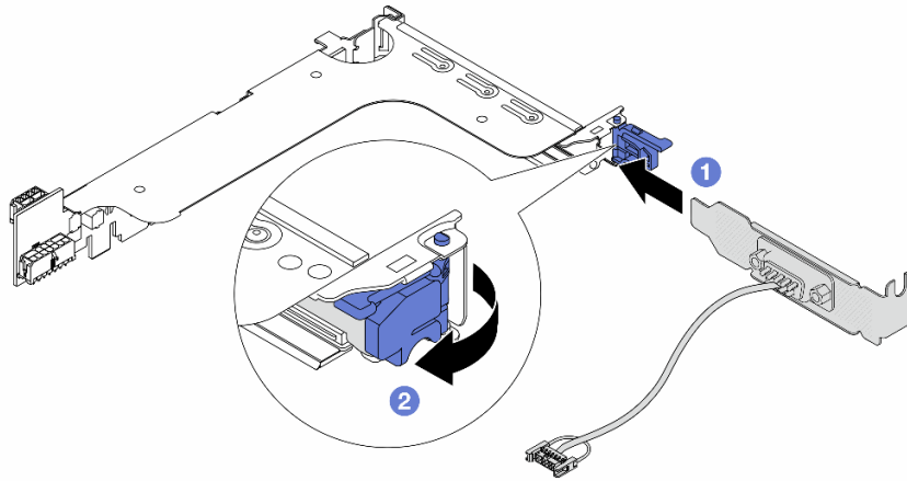
그림 251. 직렬 포트 모듈 설치
