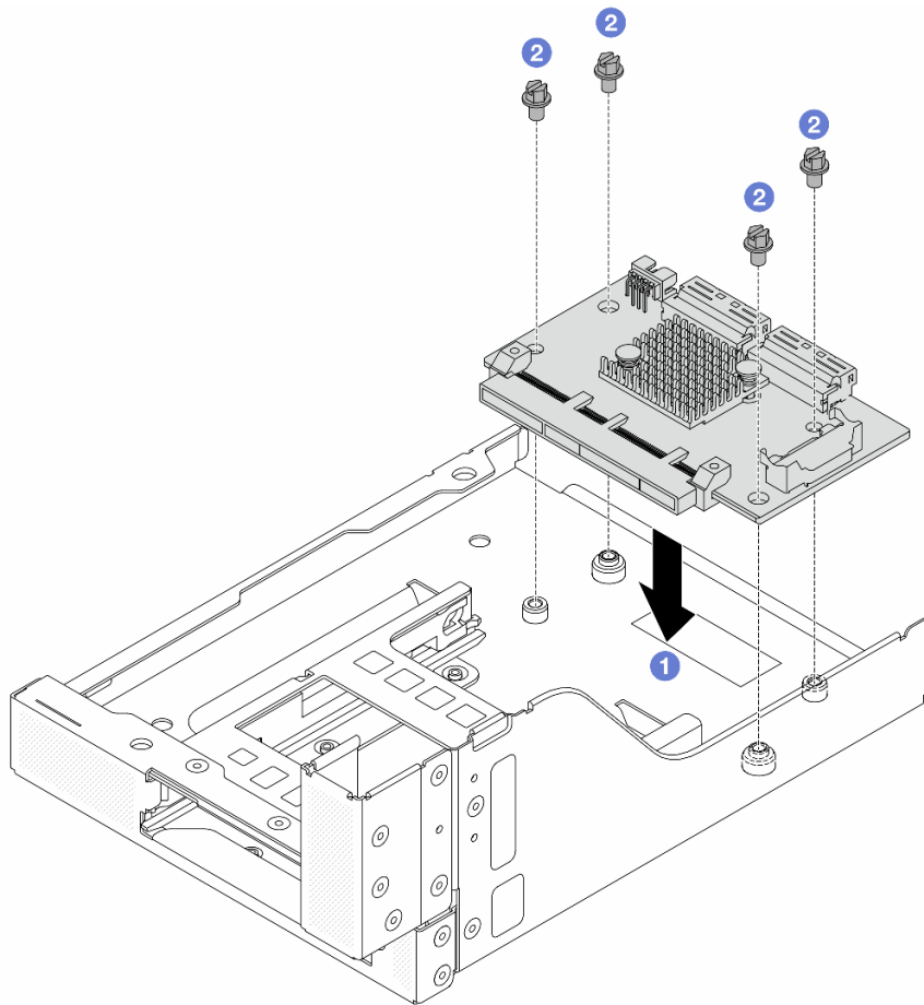
그림 51. 앞면 OCP 인터포저 카드 설치
