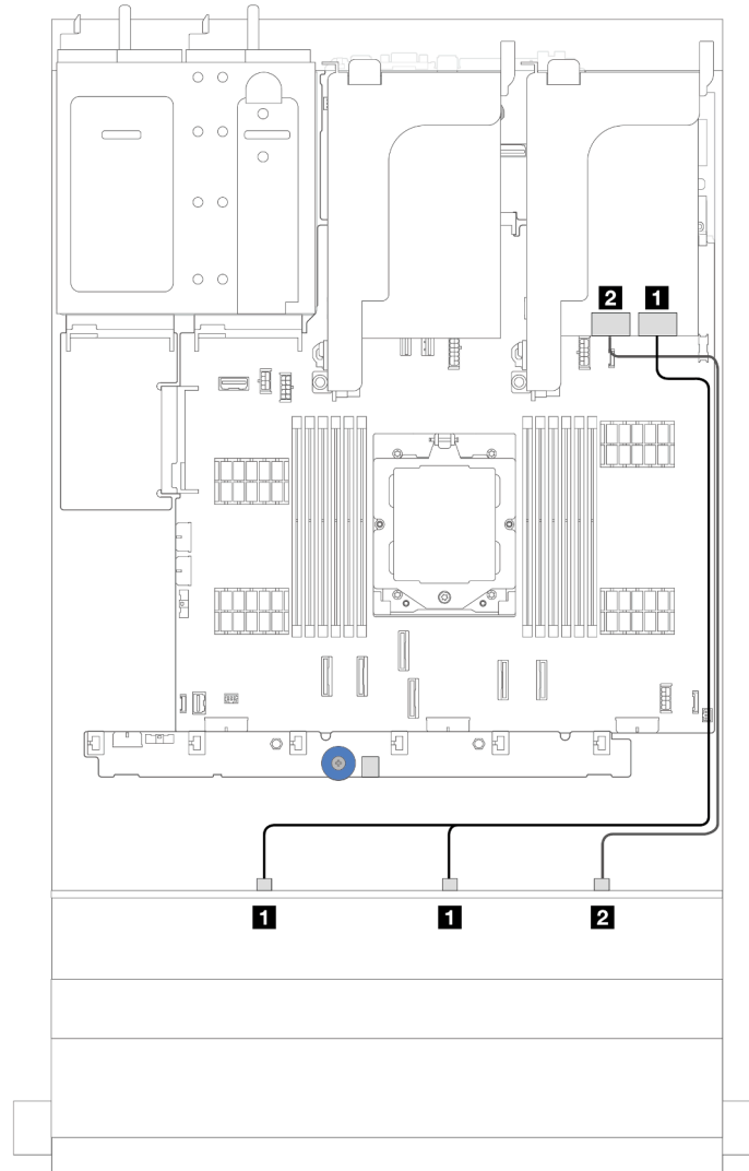
그림 387. 16i RAID/HBA 어댑터 1개가 지원되는 12 x 3.5" SAS/SATA구성의 케이블 배선
