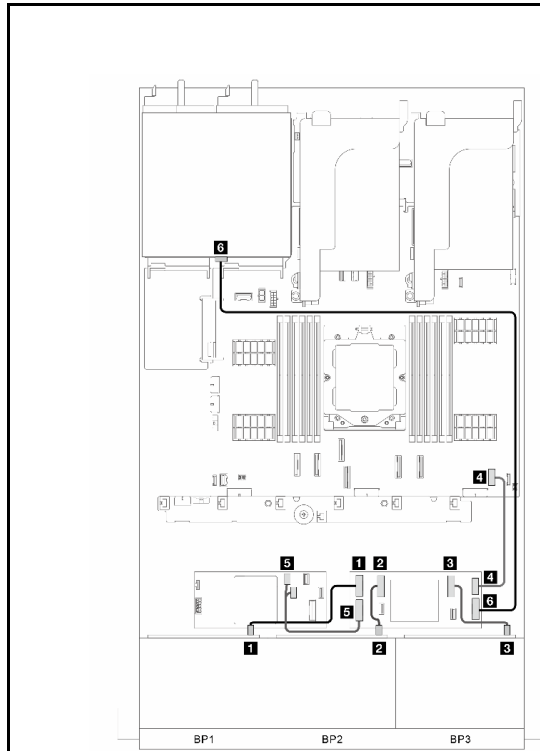
그림 344. CFF 확장기의 신호 케이블 배선
