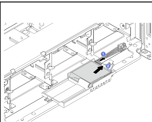
그림 180. Supercap Holder에서 RAID 플래시 전원 모듈 제거
