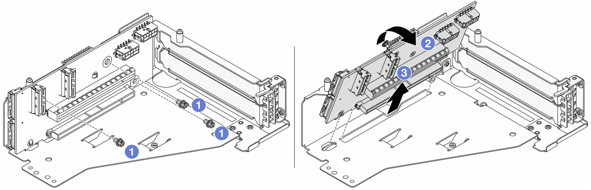
그림 36. 라이저 5 케이지에서 라이저 카드 제거
