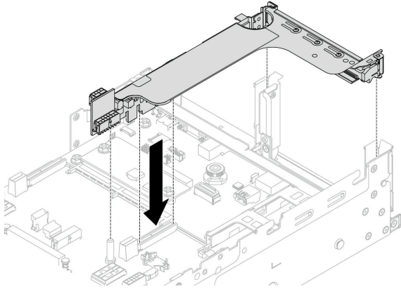
그림 252. 라이저 어셈블리 설치
