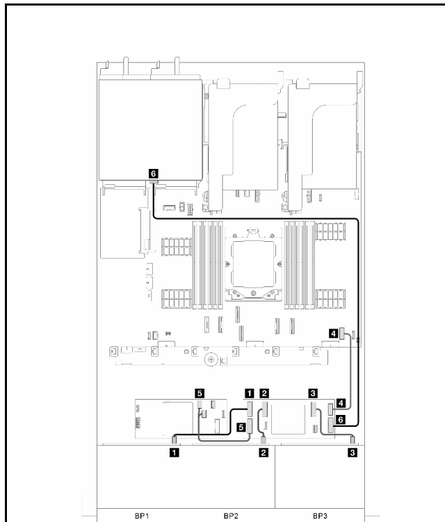
그림 339. 신호 케이블 배선 파트 1
