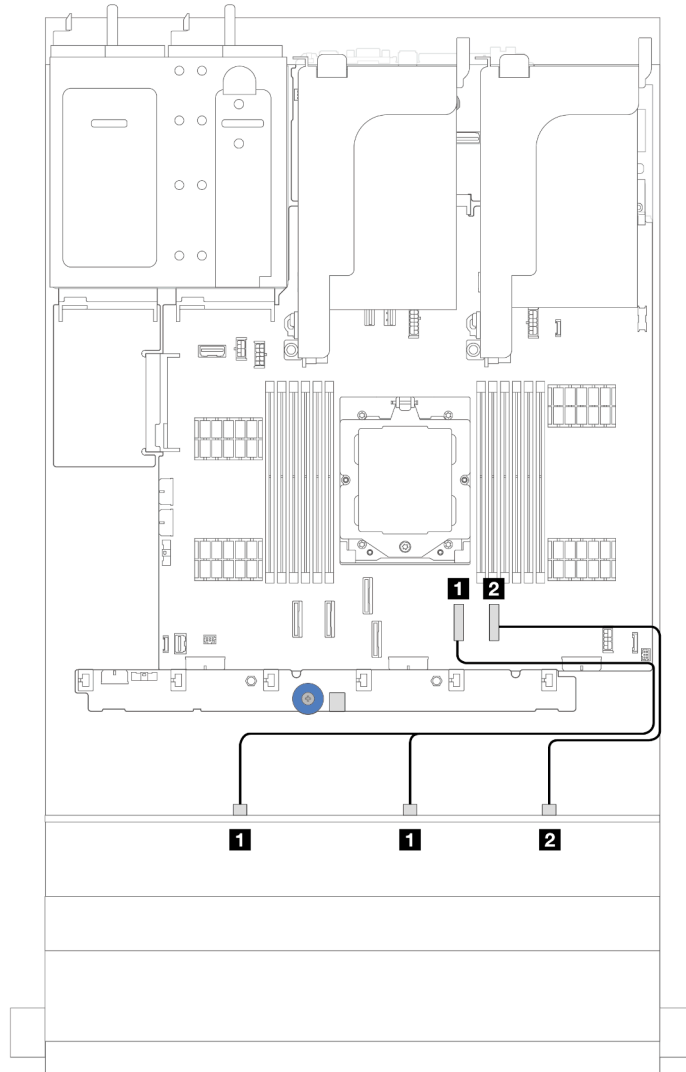
그림 386. 온보드 커넥터가 지원되는 12 x 3.5" SAS/SATA 구성의 케이블 배선
