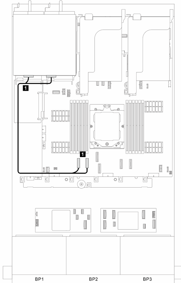
그림 343. 온보드 커넥터의 신호 케이블 배선
