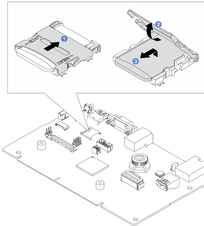
그림 122. microSD 카드 제거
