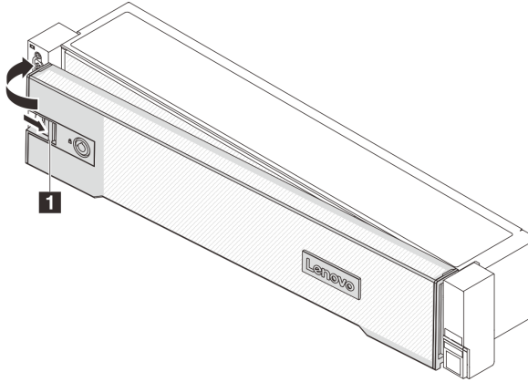
그림 233. 보안 베젤 설치
