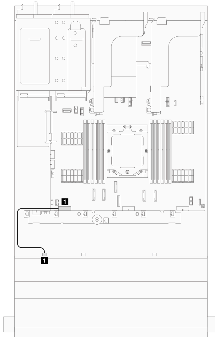
그림 372. 8 x 3.5" SAS/SATA 드라이브 백플레인의 전원 케이블 배선
