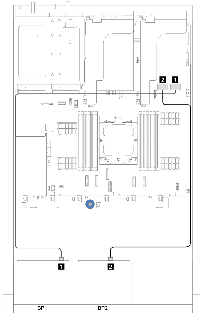
그림 320. 16i 어댑터에 대한 SAS/SATA 케이블 배선
