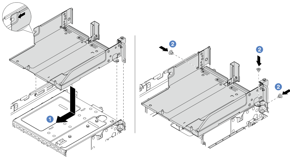
그림 148. 라이저 케이스 트레이 설치
