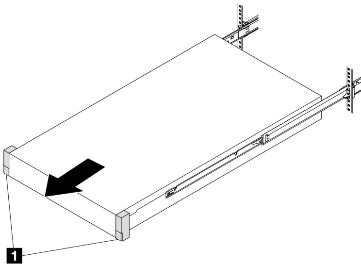
그림 18. 서버 꺼내기
