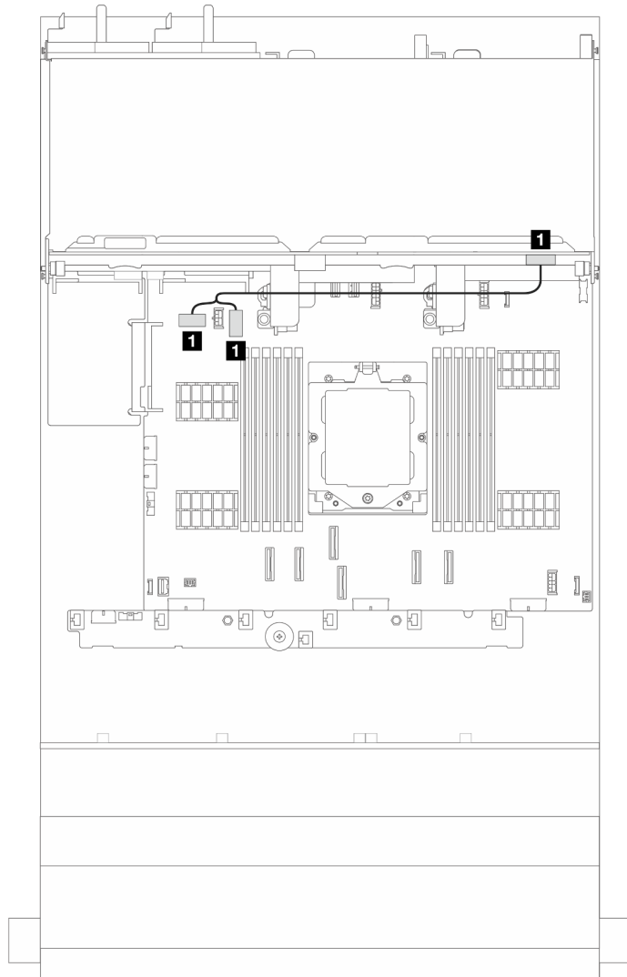
그림 376. 4 x 3.5" 뒷면 드라이브 백플레인의 전원 케이블 배선
