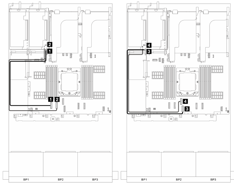
그림 298. 라이저 3/4 신호 연결
