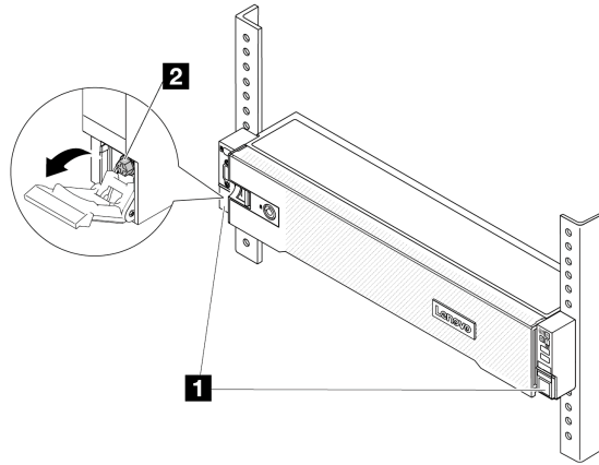
그림 17. 랙에서 서버 분리
