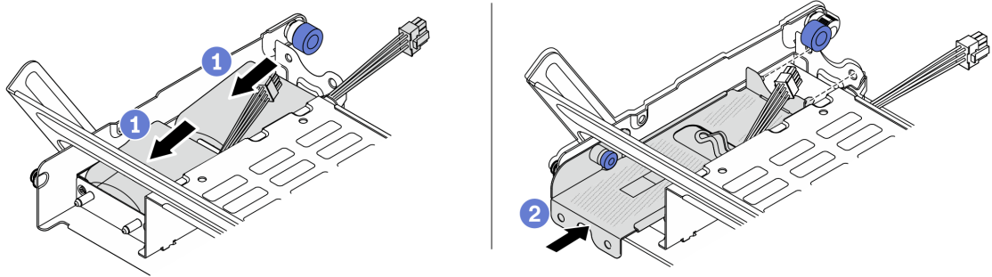
그림 192. 중간 드라이브 케이스에 RAID 플래시 전원 모듈 설치
