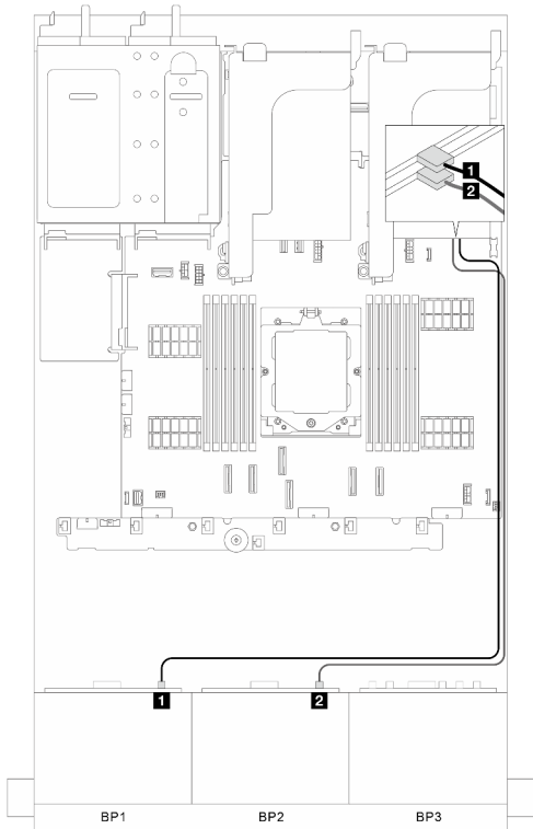
그림 333. 신호 케이블 배선 파트 1
