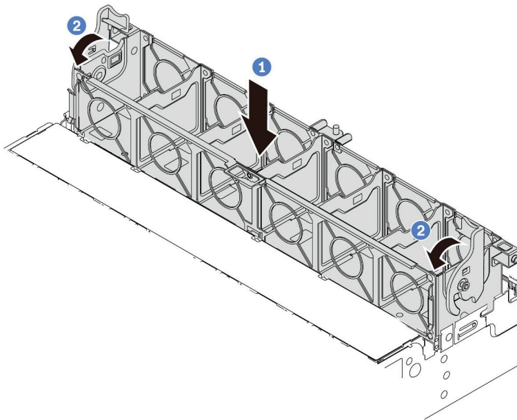
그림 245. 시스템 팬 케이스 설치
