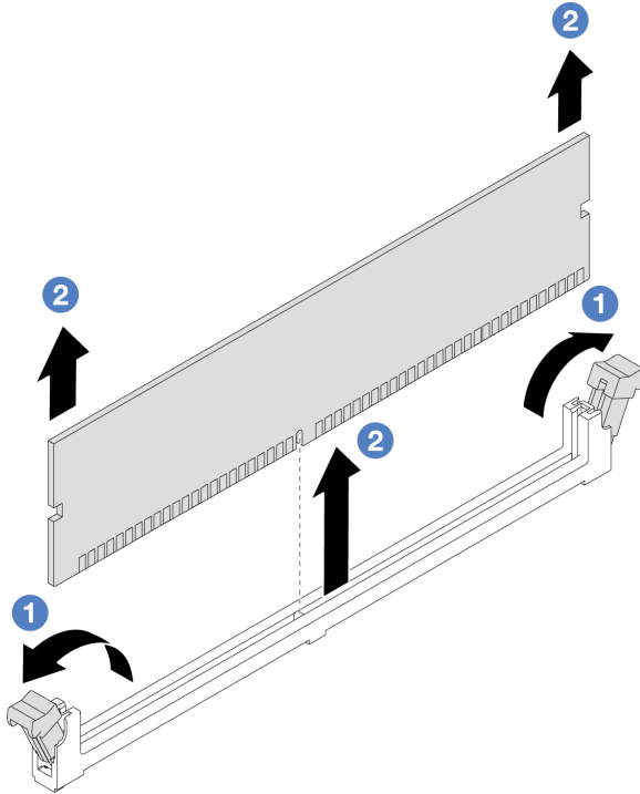
그림 120. 메모리 모듈 제거
