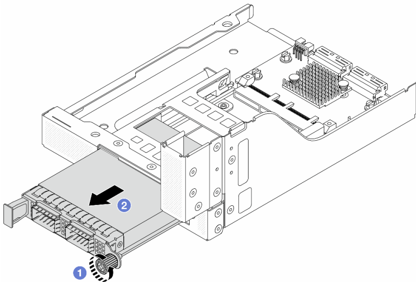
그림 49. OCP 모듈 제거
