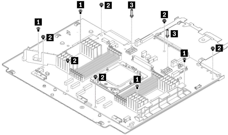
그림 411. 프로세서 보드에서 나사 제거
