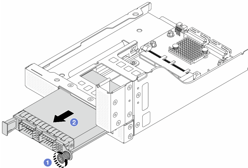
그림 37. OCP 모듈 제거
