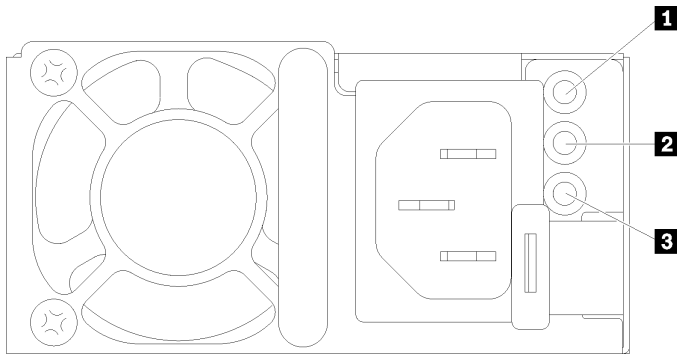
그림 407. 전원 공급 장치 LED
