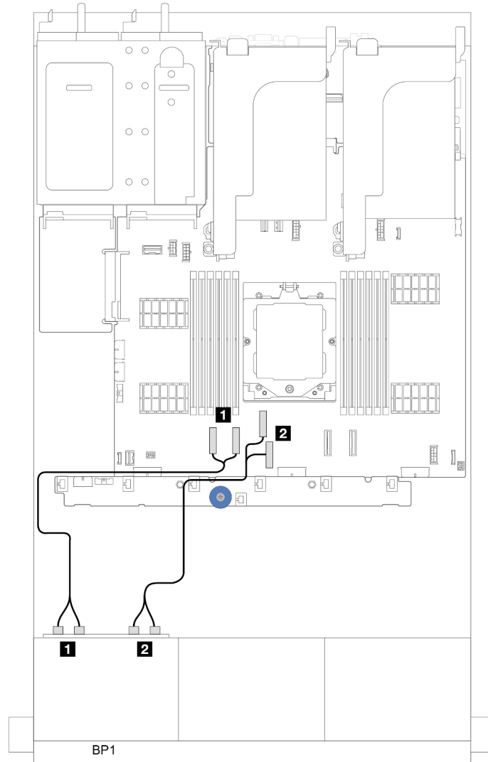
그림 309. 프로세서 1개가 설치된 경우 케이블 배선
