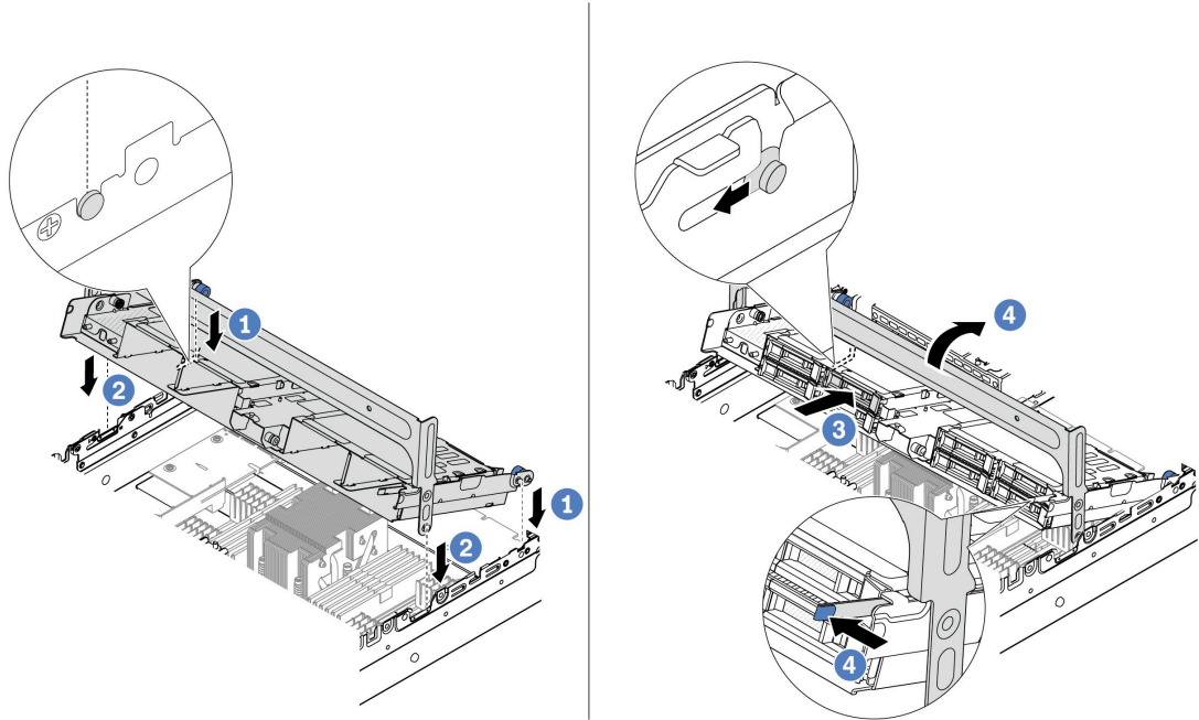
그림 129. 중간 드라이브 케이지 및 드라이브 설치
