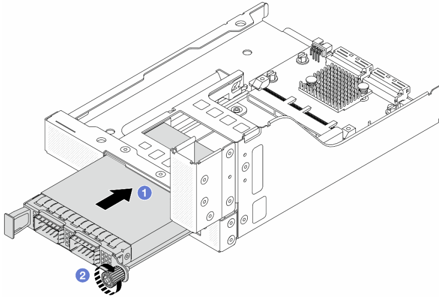
그림 52. OCP 모듈 설치
