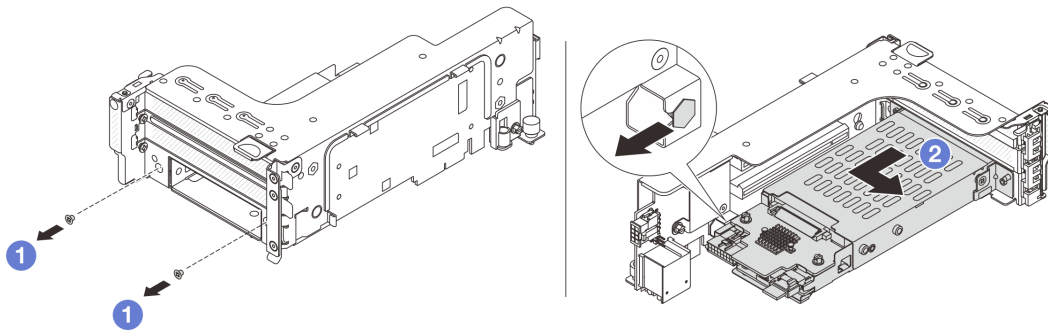
그림 203. 라이저 어셈블리에서 7mm 드라이브 케이스 제거
