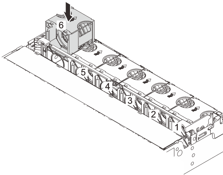
그림 243. 시스템 팬 설치
