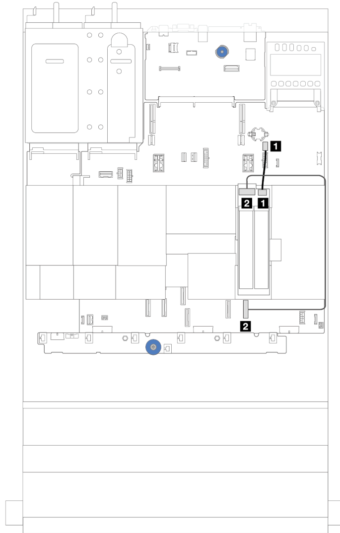
그림 283. M.2 드라이브 백플레인의 SATA/NVMe 케이블 배선
