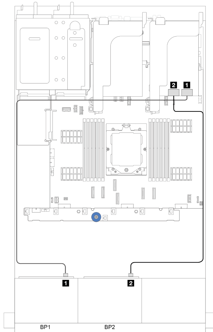
그림 316. 16i RAID/HBA 어댑터에 대한 SAS/SATA 케이블 배선
