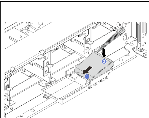
그림 186. Supercap Holder에 RAID 플래시 전원 모듈 설치
