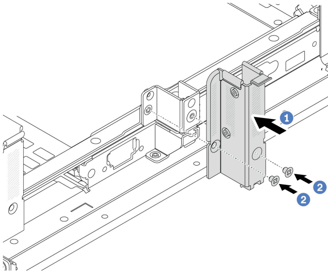
그림 199. B1 뒷면 벽 브래킷 설치(중간)
