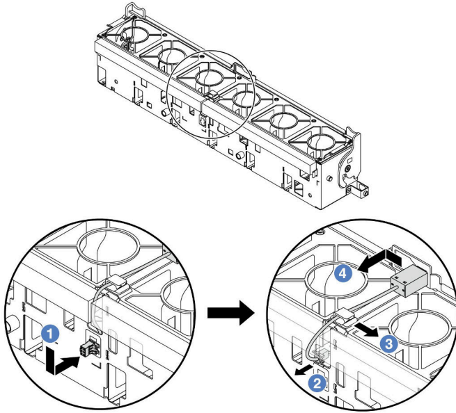
그림 102. 침입 스위치 제거
