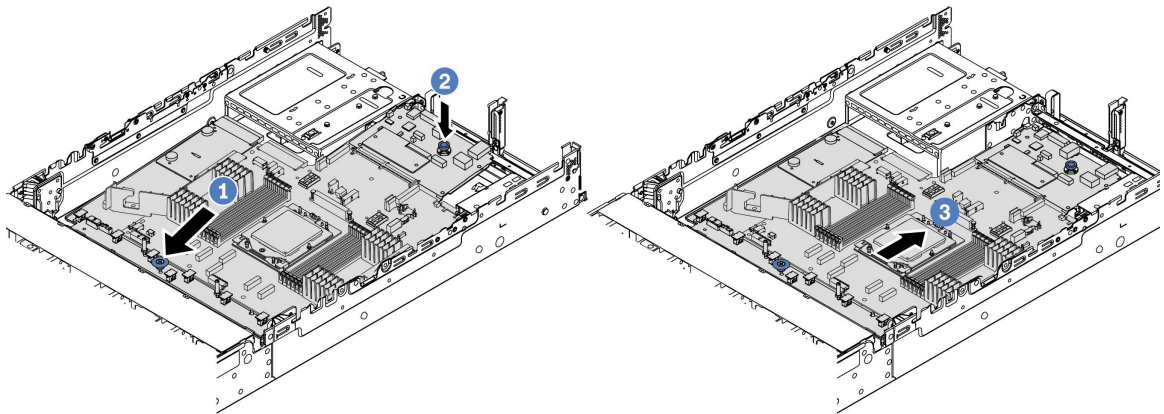
그림 241. 시스템 보드 어셈블리 설치
