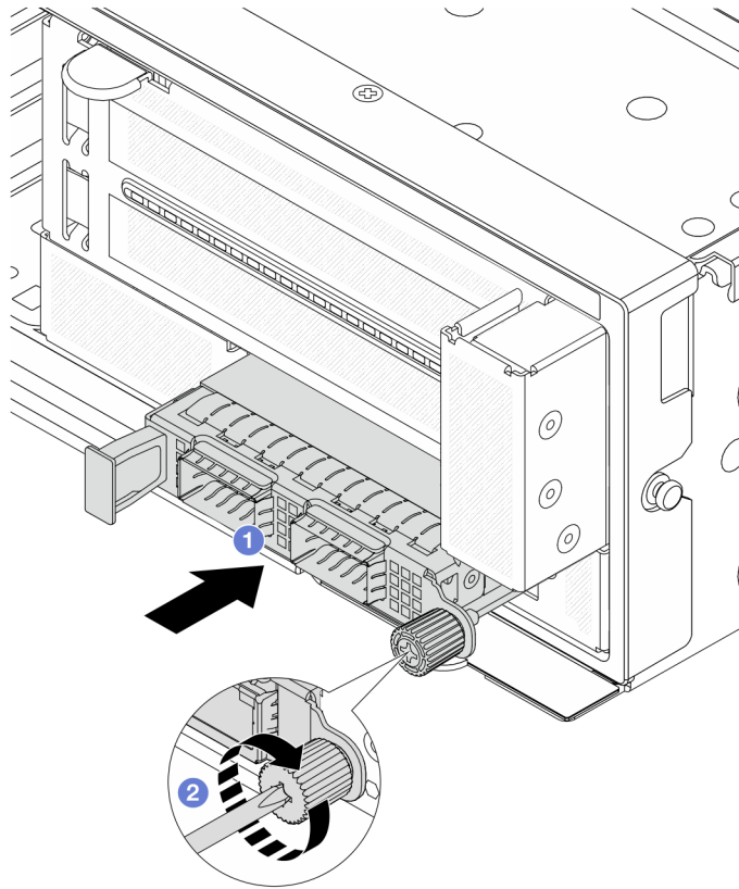
그림 46. 앞면 OCP 모듈 설치
