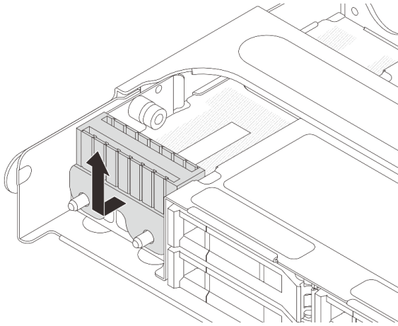
그림 189. 고무 제거
