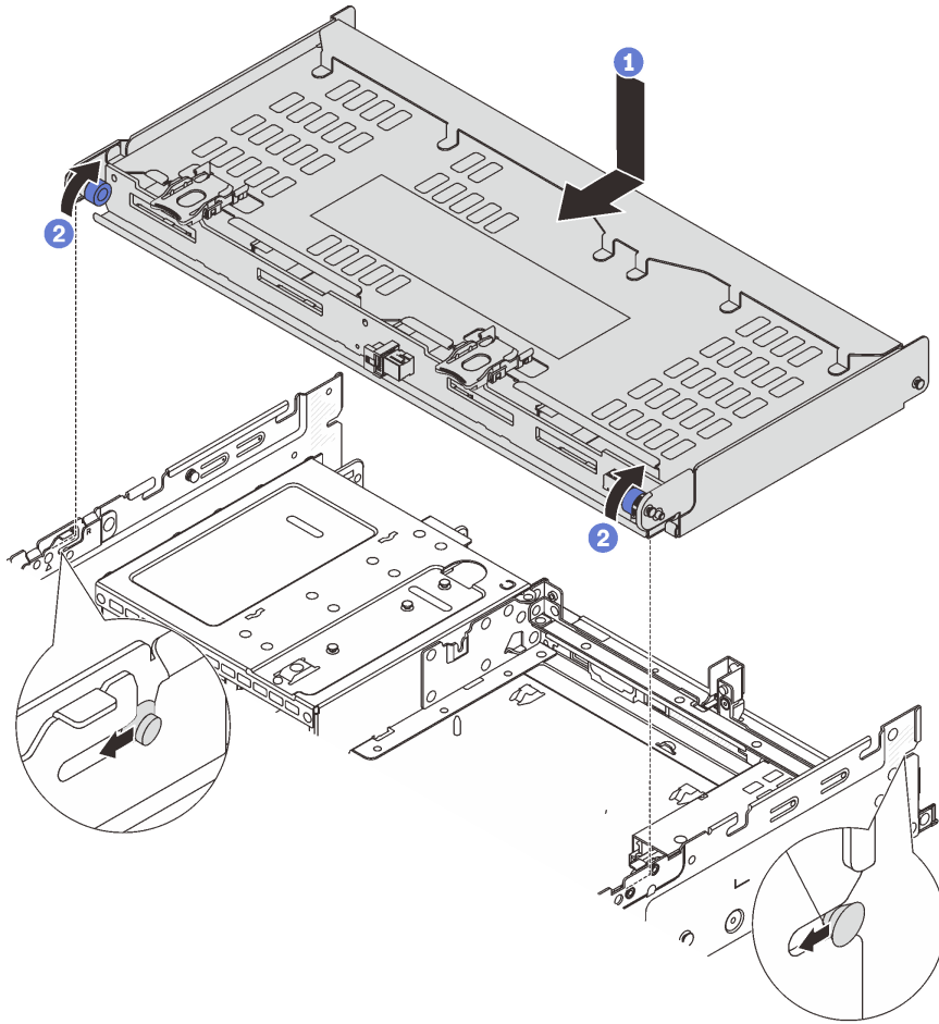
그림 228. 4 x 3.5" 뒷면 드라이브 케이지 설치
