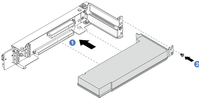
그림 145. 4LP 라이저 3/4 어셈블리에 PCIe 어댑터 설치
