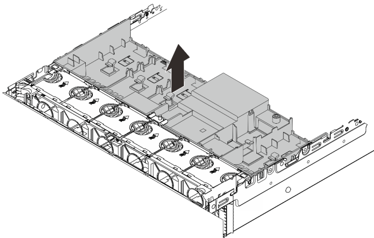
그림 27. 공기 조절 장치 제거
