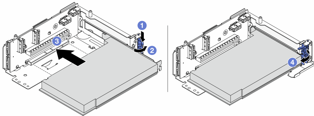
그림 62. 라이저 5 케이스에 PCIe 어댑터 설치
