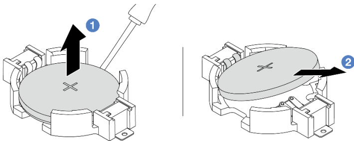
그림 31. CMOS 배터리 제거
