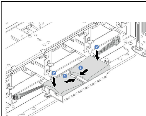
그림 185. Supercap Holder에 RAID 플래시 전원 모듈 설치
