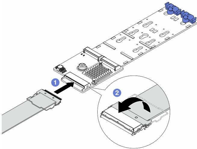
그림 117. ThinkSystem M.2 RAID B540i-2i SATA/NVMe Enablement Kit에 M.2 케이블 연결
