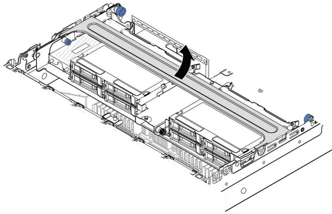
그림 190. 중간 드라이브 케이지의 손잡이 열기
