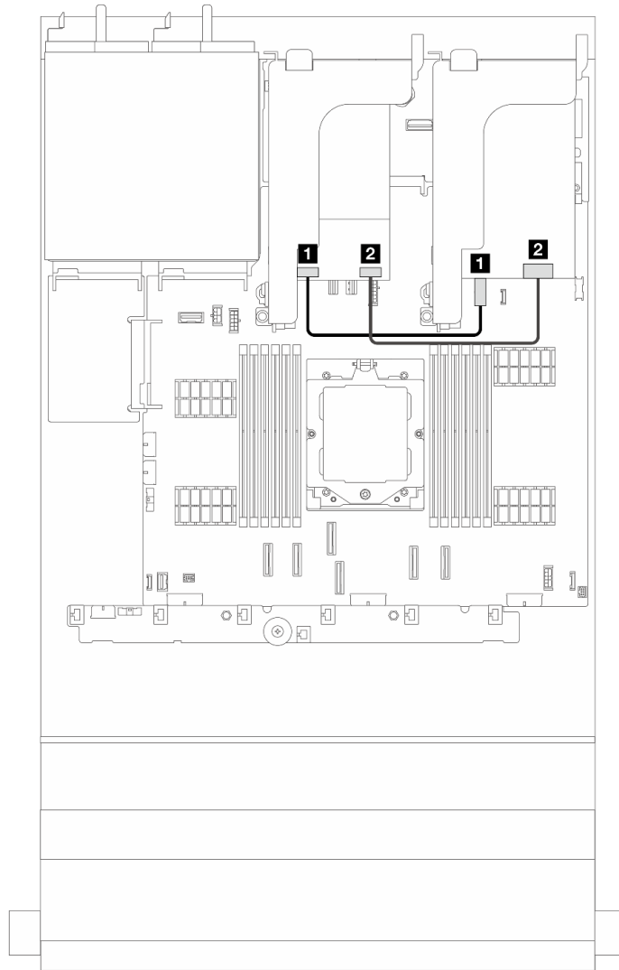
그림 272. 7mm 드라이브 백플레인의 RAID 케이블 배선
