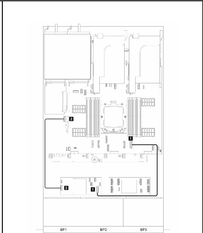
그림 351. 신호 케이블 배선 파트 2
