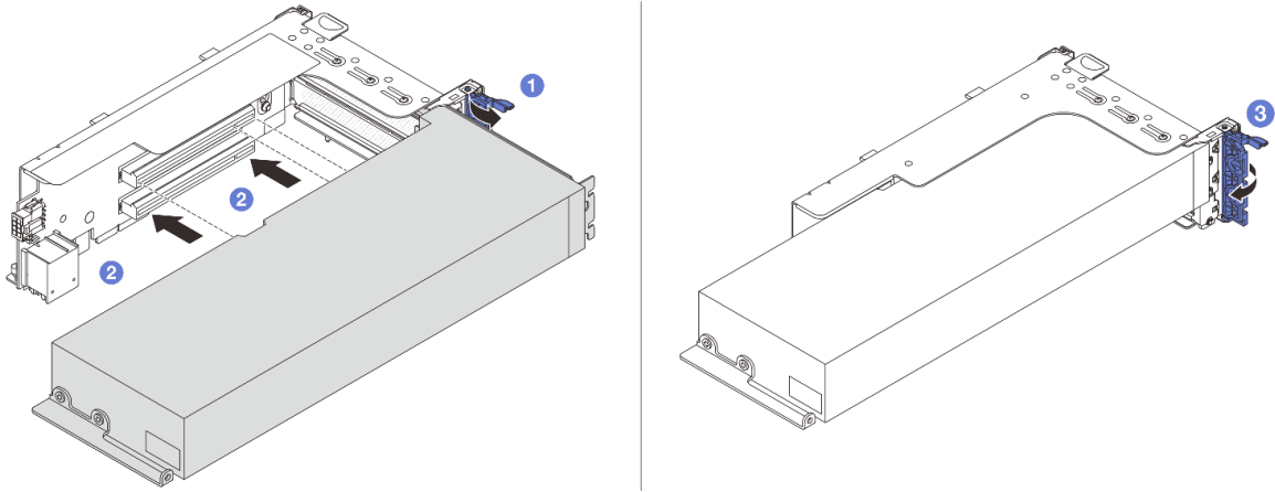
그림 88. GPU 어댑터 설치
