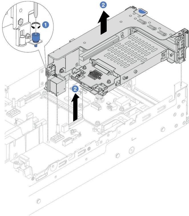
그림 201. 2FH+7mm SSD 라이저 케이지 제거
