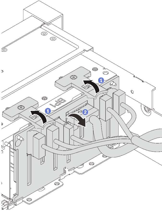
그림 67. 2.5" 드라이브 백플레인 제거
