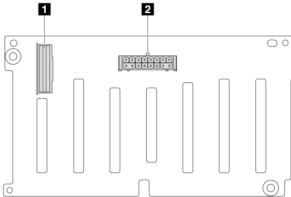
그림 256. 8 x 2.5" SAS/SATA 백플레인 커넥터
