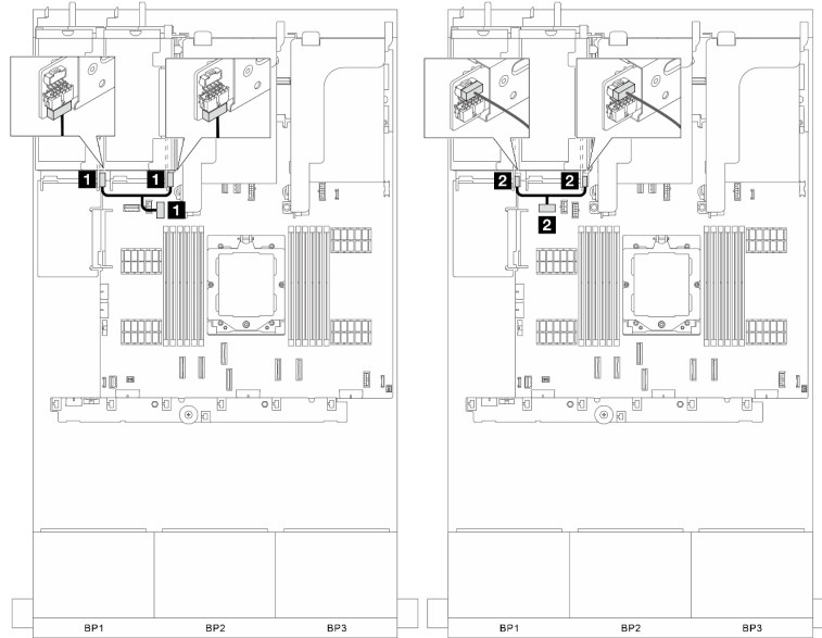
그림 297. 라이저 3/4 전원 및 사이드밴드 연결
