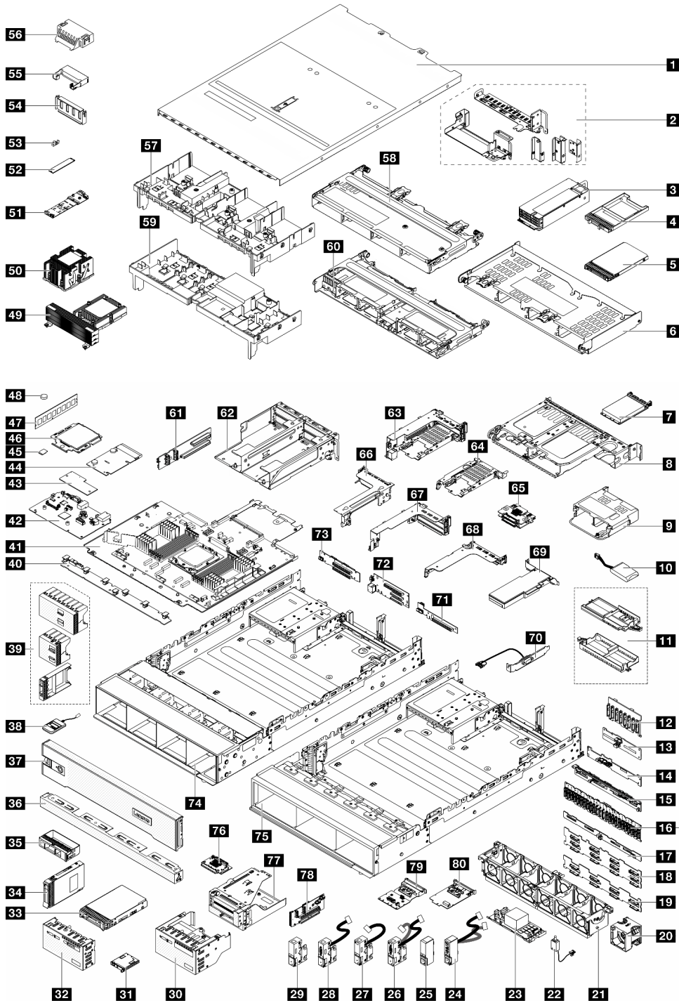
그림 13. 서버 구성 요소
