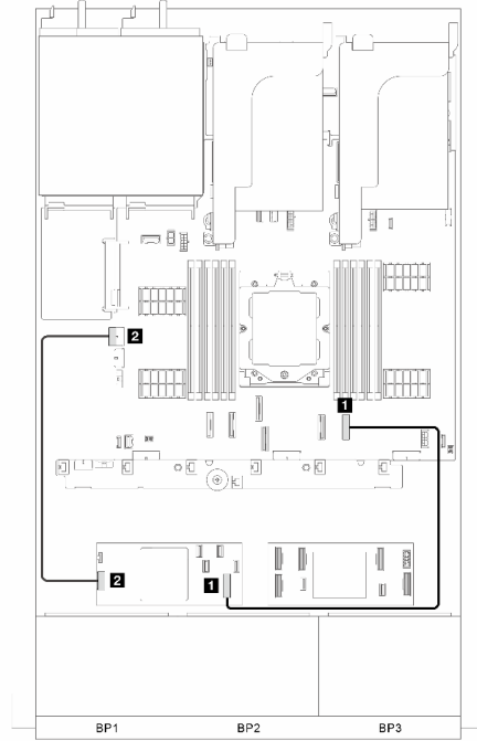
그림 357. 신호 케이블 배선 파트 2
