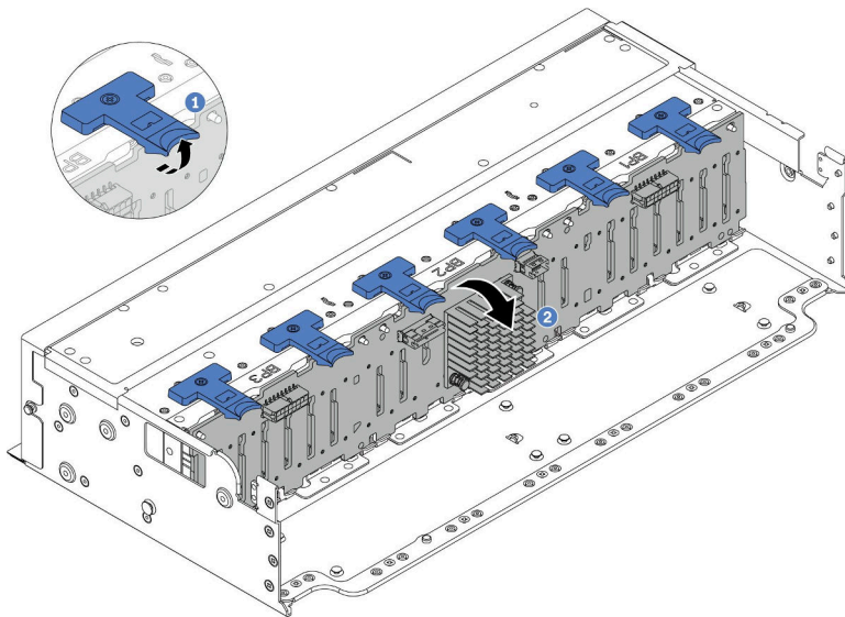
그림 68. 24베이 드라이브 백플레인 제거
