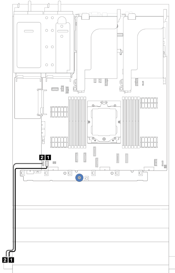
그림 269. 앞면 VGA 커넥터 및 외부 진단 커넥터의 케이블 배선
