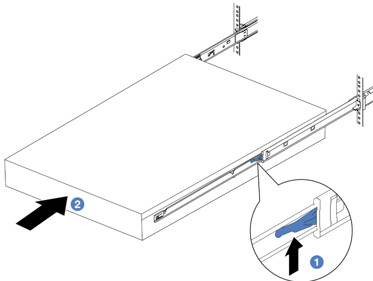
그림 24. 랙에 서버 설치
