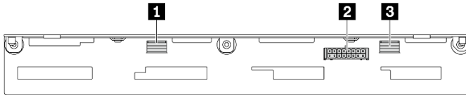
그림 267. 8x2.5" SAS/SATA 백플레인 커넥터
