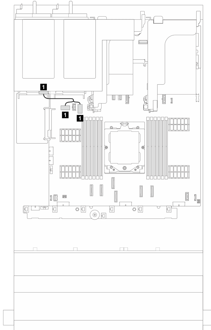
그림 304. 뒷면 드라이브 백플레인의 전원 케이블 연결
