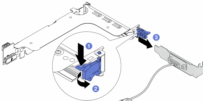
그림 248. 직렬 포트 모듈 제거
