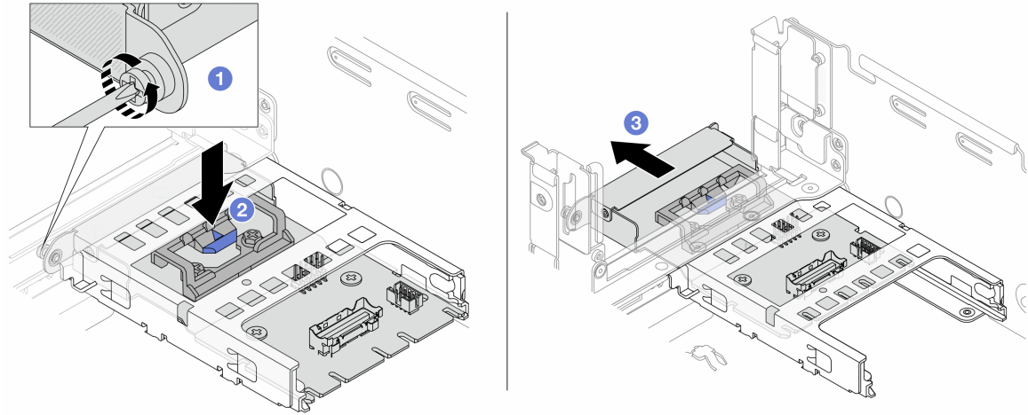
그림 55. 뒷면 OCP 인터포저 카드 제거
