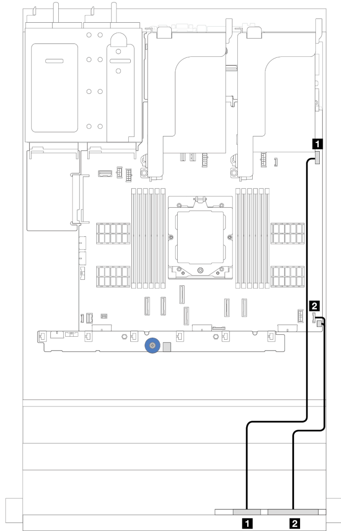
그림 277. 미디어 베이의 내장형 진단 패널용 케이블 배선
