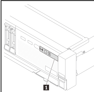
1 LCD 디스플레이가 없는 앞면 오퍼레이터 패널
