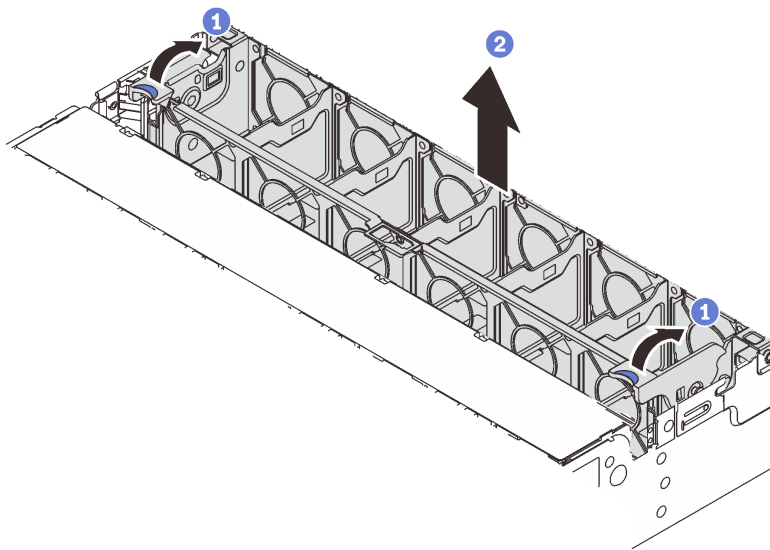
그림 244. 시스템 팬 케이스 제거
