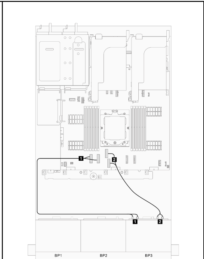
그림 330. 신호 케이블 배선 파트 2
