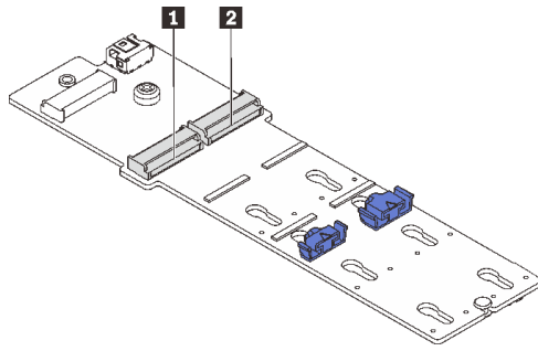
그림 106. M.2 드라이브 슬롯
