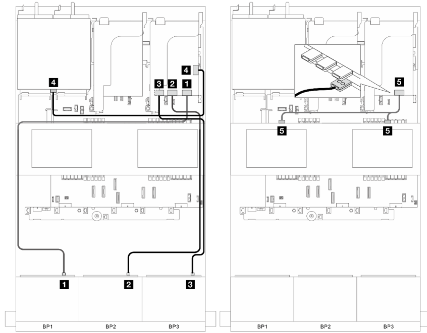
그림 355. 신호 케이블 배선
