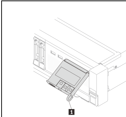
그림 5. 내장형 진단 패널(LCD 디스플레이 포함)
