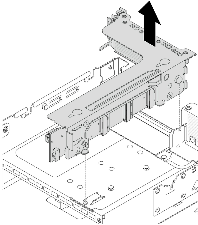
그림 131. 라이저 3 어셈블리 제거
