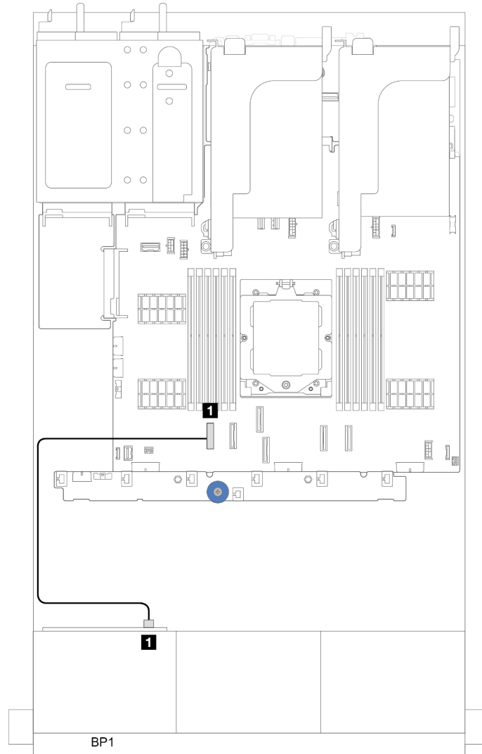
그림 311. 프로세서 1개가 설치된 경우 케이블 배선
