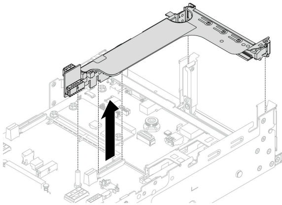
그림 247. 라이저 브래킷 제거
