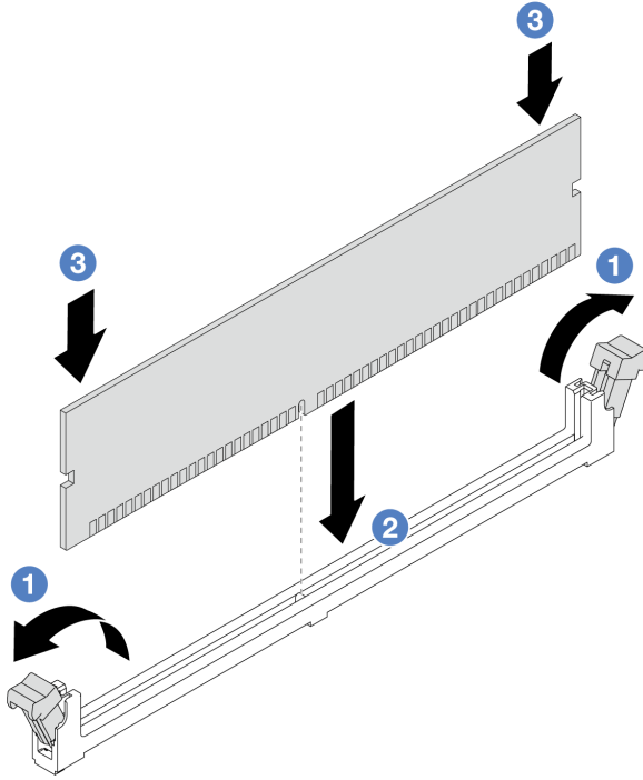
그림 121. 메모리 모듈 설치
