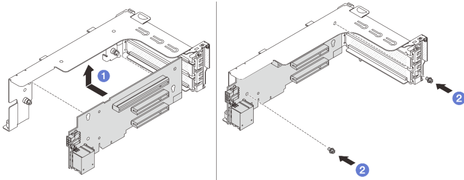
그림 140. 라이저 카드 1 설치
