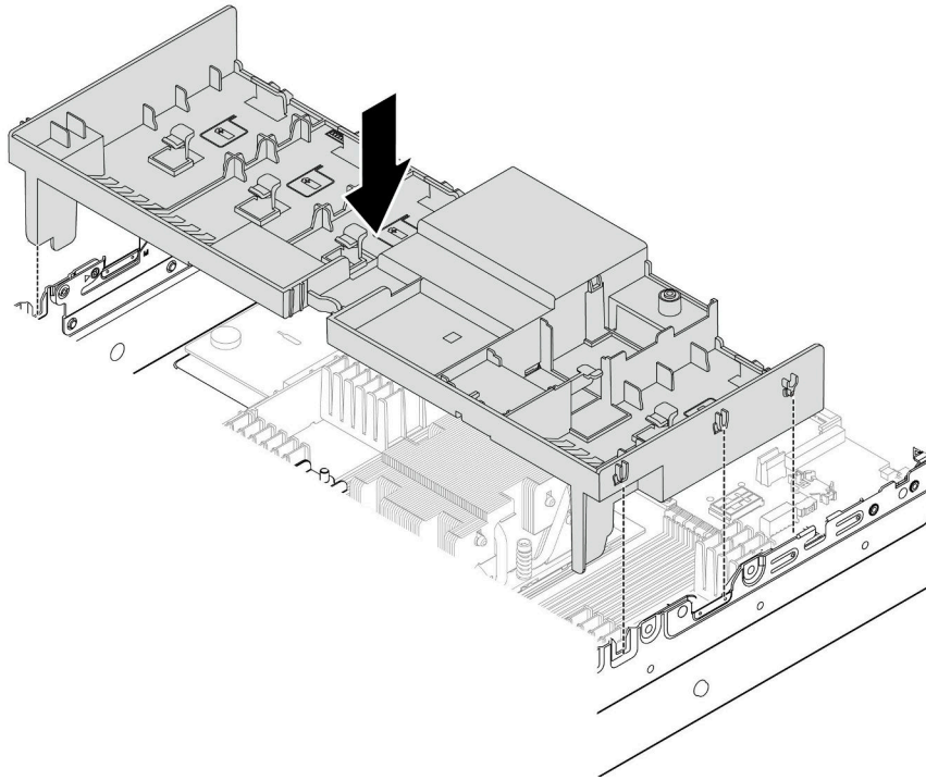
그림 30. 공기 조절 장치 설치
