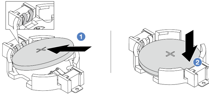
그림 32. CMOS 배터리 설치
