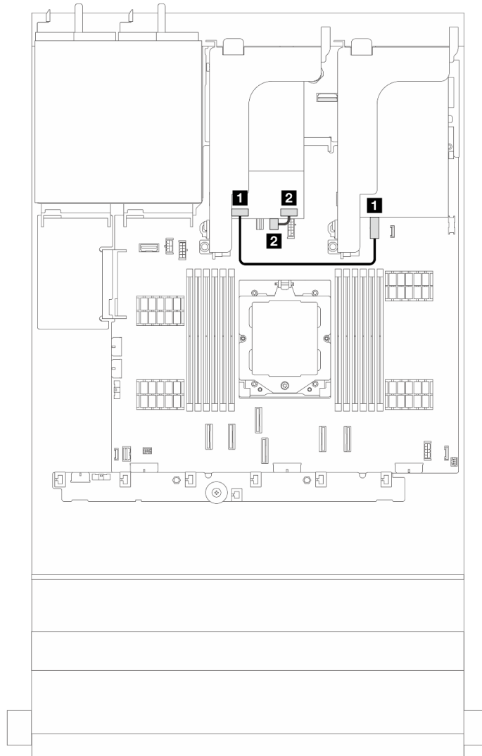
그림 274. 7mm 드라이브 백플레인의 케이블 배선
