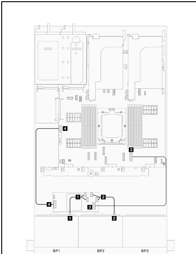
그림 327. 신호 케이블 배선 파트 1
