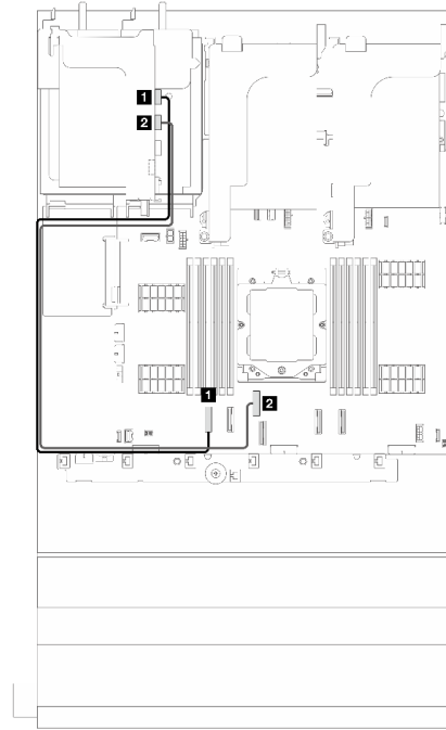
그림 296. 라이저 3(x8/x8 Gen 4) 신호 케이블 배선
