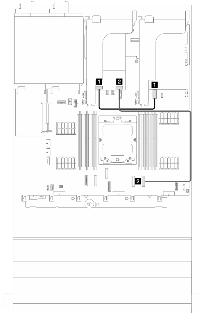
그림 270. 7mm 드라이브 백플레인의 SATA 케이블 배선
