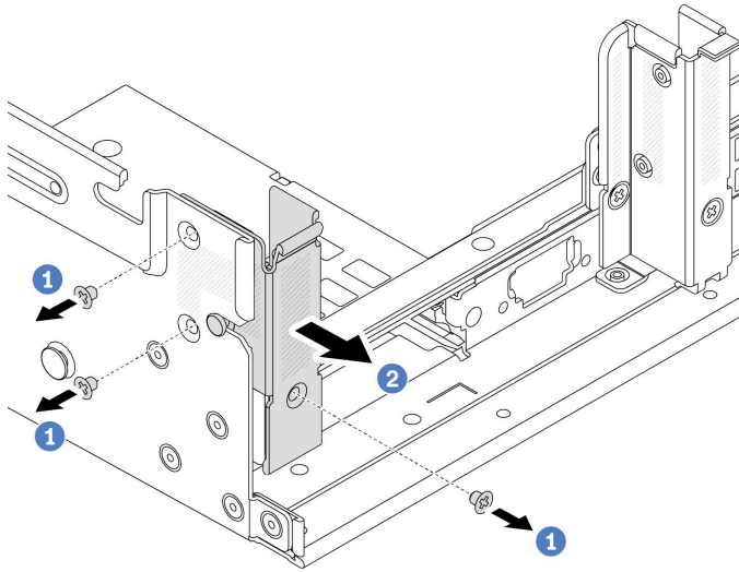
그림 195. A1 뒷면 벽 브래킷 제거(왼쪽)
