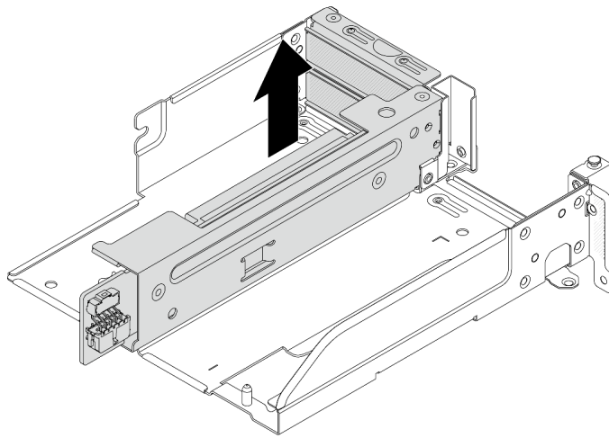
그림 132. 라이저 3/4 어셈블리 제거
