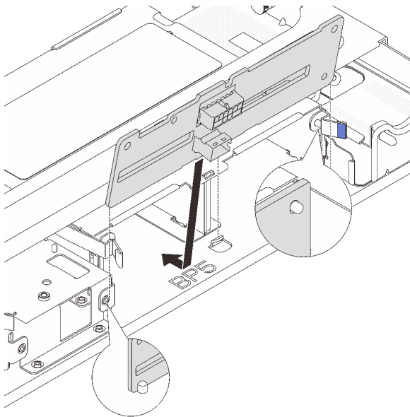
그림 127. 중간 2.5" 드라이브 백플레인 설치
