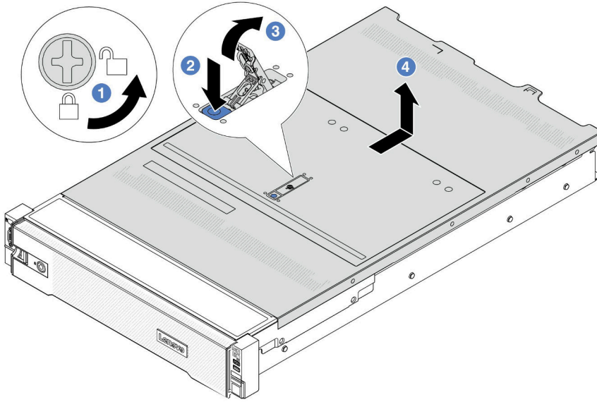
그림 253. 윗면 덮개 제거
