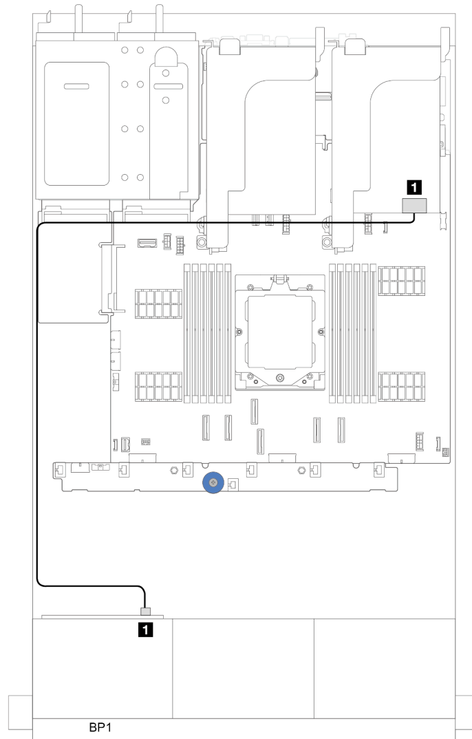
그림 313. 8i/16i RAID/HBA 어댑터에 대한 SAS/SATA 케이블 배선
