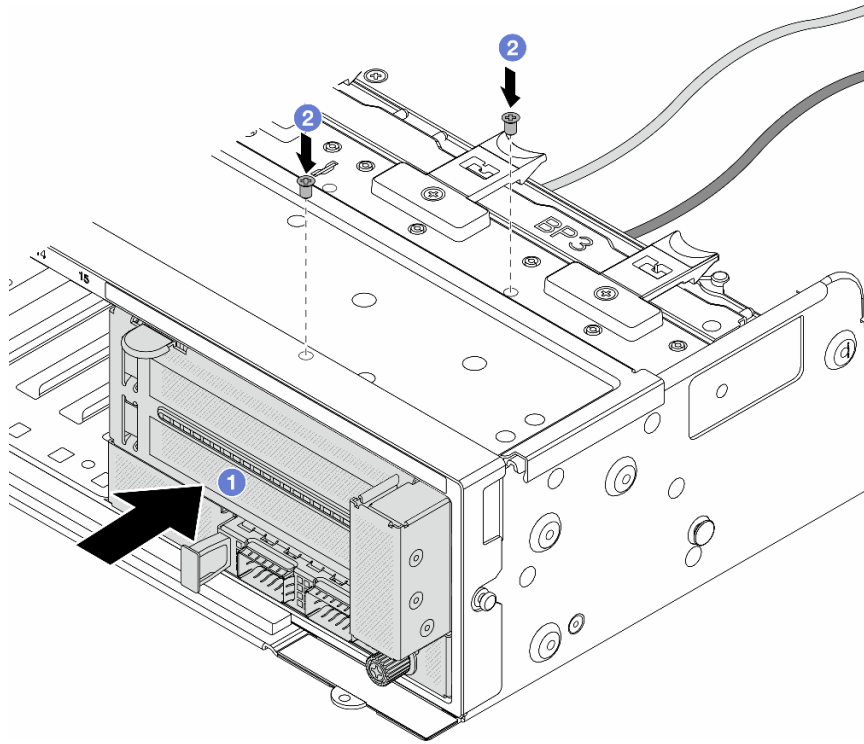
그림 54. 앞면 어댑터 어셈블리 설치
