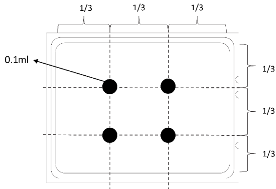
그림 165. 열전도 그리스 도포
