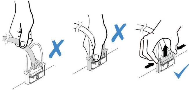
그림 246. 시스템 I/O 보드에서 케이블 분리
