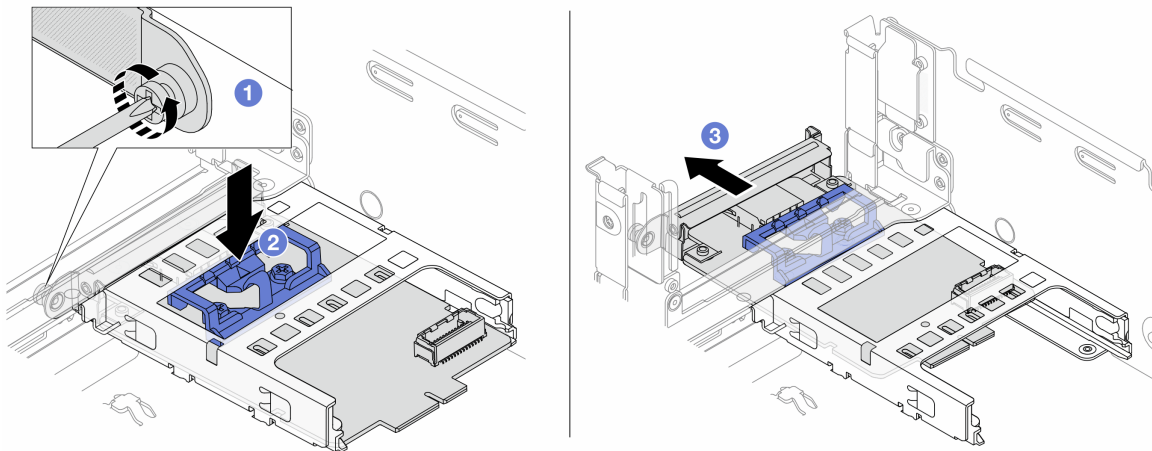
그림 118. 관리 NIC 어댑터 제거
