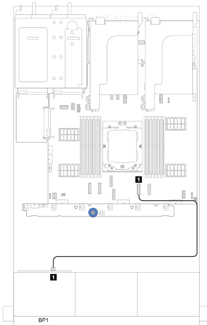
그림 310. 온보드 SATA 커넥터에 대한 SAS/SATA 케이블 배선
