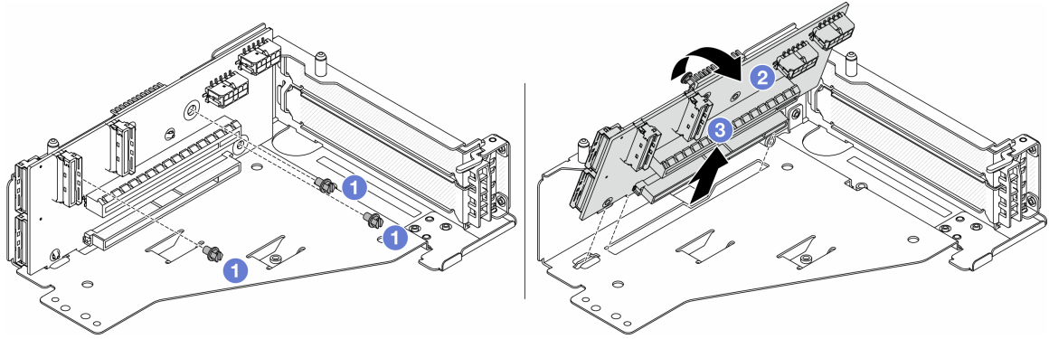
그림 60. 라이저 5 케이스에서 라이저 카드 제거
