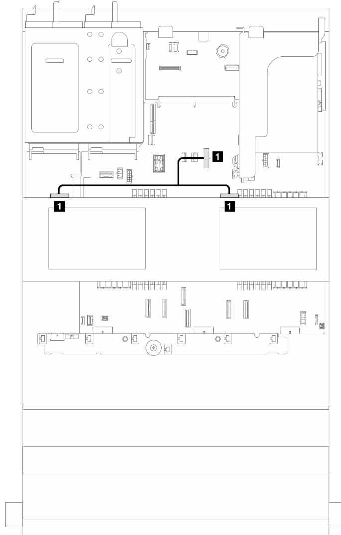
그림 378. 4 x 2.5" 중간 드라이브 백플레인 2개의 전원 케이블 배선
