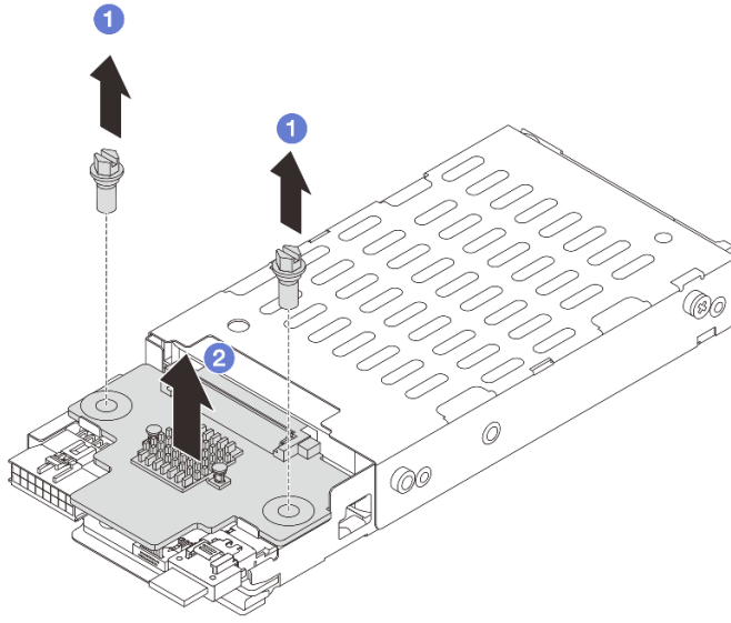
그림 205. 7mm 드라이브 백플레인 제거(상단)
