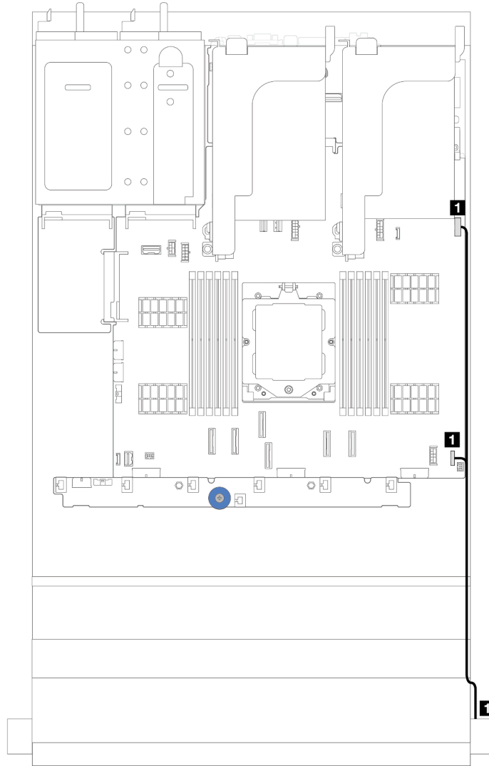
그림 276. 오른쪽 랙 래치의 앞면 I/O 모듈에 대한 케이블 배선
