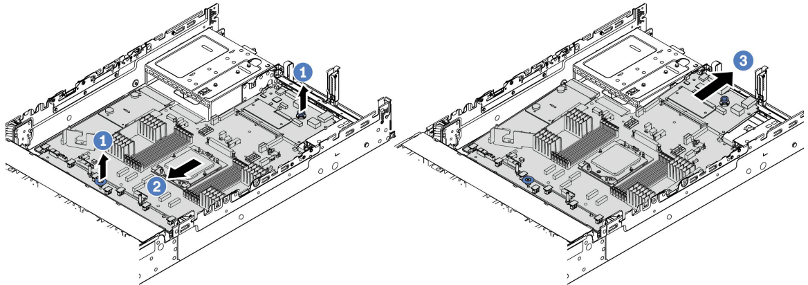
그림 238. 시스템 보드 어셈블리 제거
