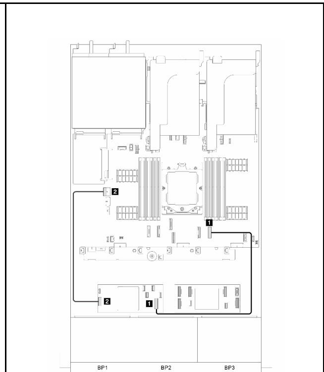
그림 340. 신호 케이블 배선 파트 2
