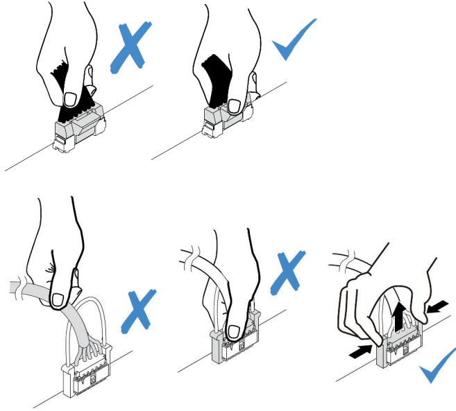
그림 76. 시스템 보드 어셈블리에서 케이블 분리
