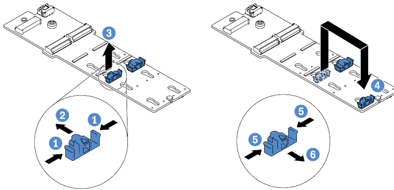
그림 105. M.2 고정장치 조정
