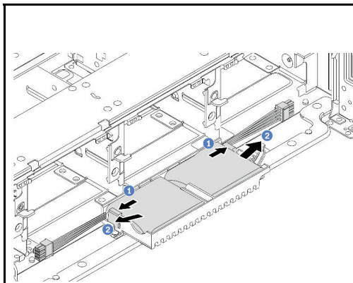
그림 179. Supercap Holder에서 RAID 플래시 전원 모듈 제거
