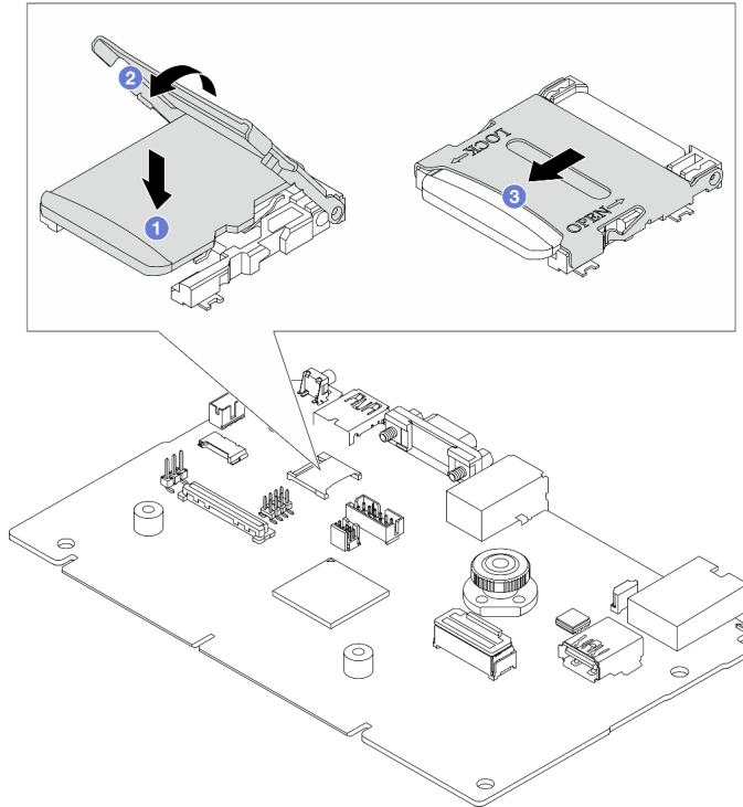
그림 123. MicroSD 카드 설치
