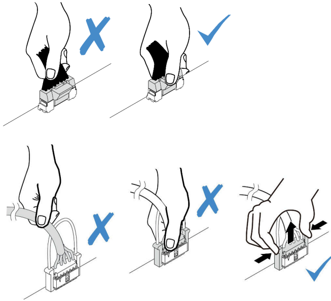
그림 168. 시스템 보드 어셈블리에서 케이블 분리
