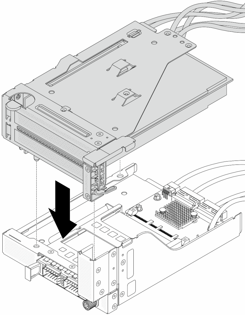
그림 63. 앞면 OCP 어셈블리에 라이저 5 어셈블리 설치
