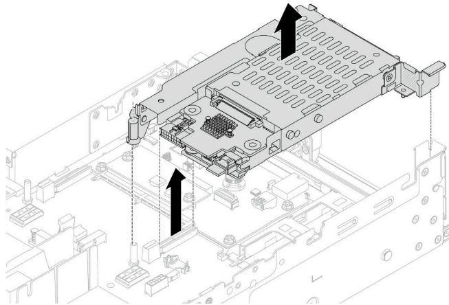
그림 202. 7mm SSD 라이저 케이스 제거
