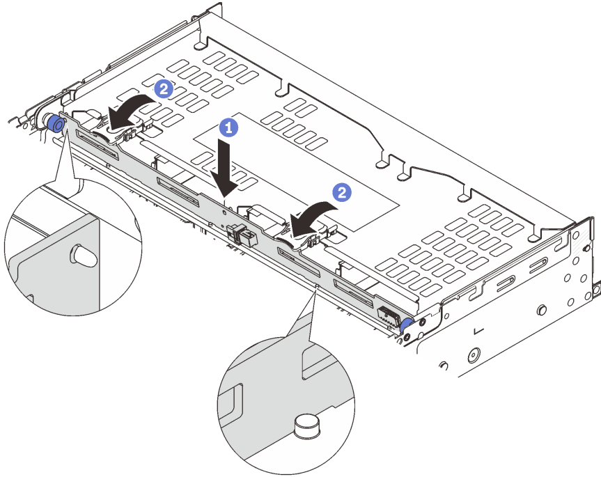
그림 227. 4 x 3.5" 뒷면 드라이브 백플레인 설치
