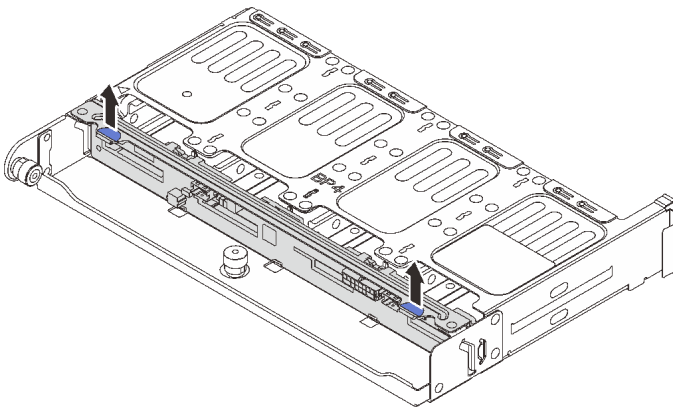
그림 218. 뒷면 8 x 2.5" 드라이브 백플레인 제거
