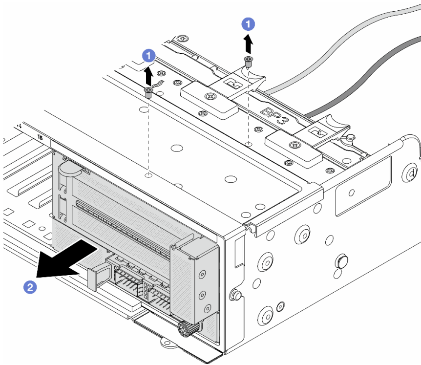
그림 57. 전면 어댑터 어셈블리 제거
