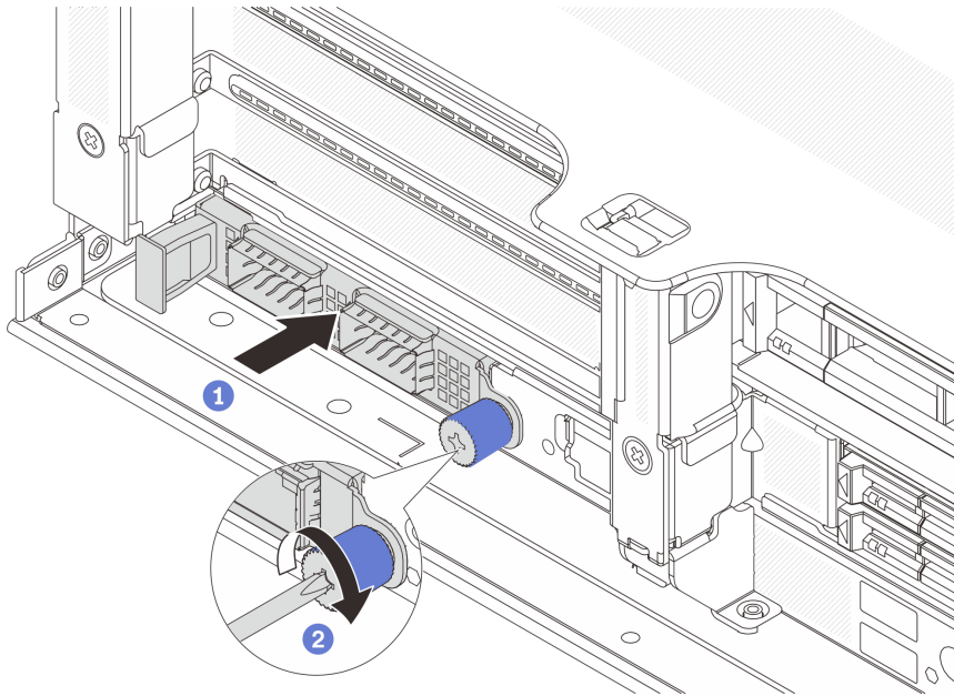
그림 151. OCP 뒷면 모듈 설치
