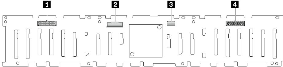
그림 258. 24 x 2.5" SAS/SATA 확장기 백플레인의 커넥터
