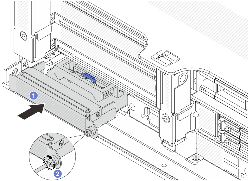
그림 56. 뒷면 OCP 인터포저 카드 설치
