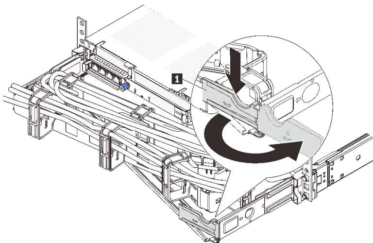
그림 156. CMA 조정
