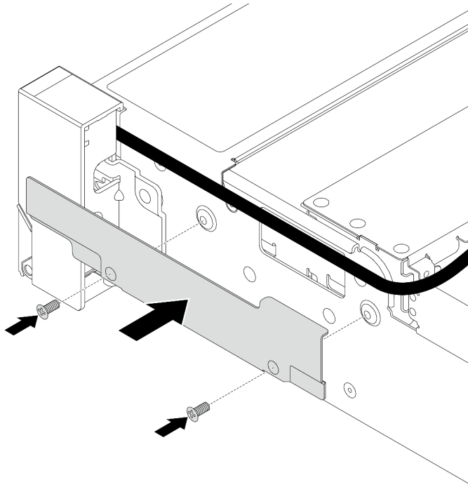
그림 174. 케이블 고정장치 설치
