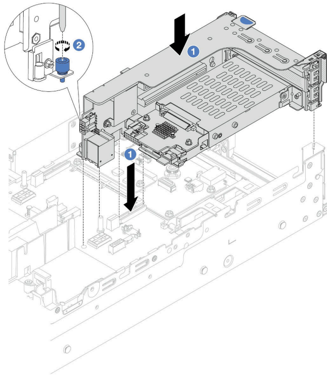
그림 211. 2FH+7mm SSD 라이저 케이스 설치
