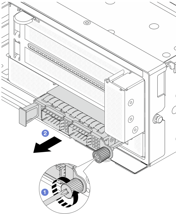
그림 45. 앞면 OCP 모듈 제거
