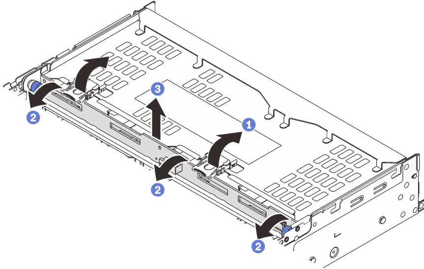
그림 226. 4 x 3.5" 뒷면 드라이브 백플레인 제거
