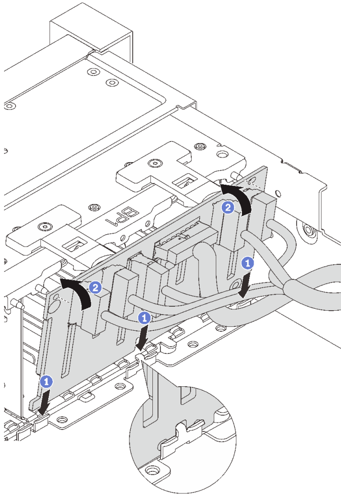
그림 70. 2.5" 드라이브 백플레인 설치
