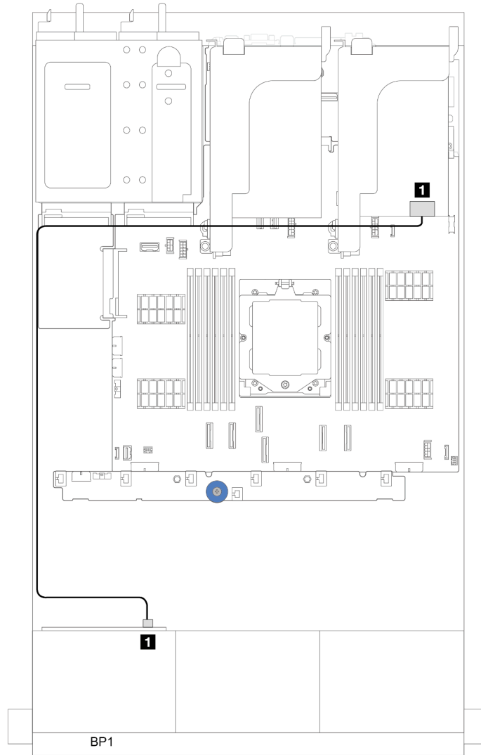
그림 306. 8i/16i RAID/HBA 어댑터에 대한 SAS/SATA 케이블 배선
