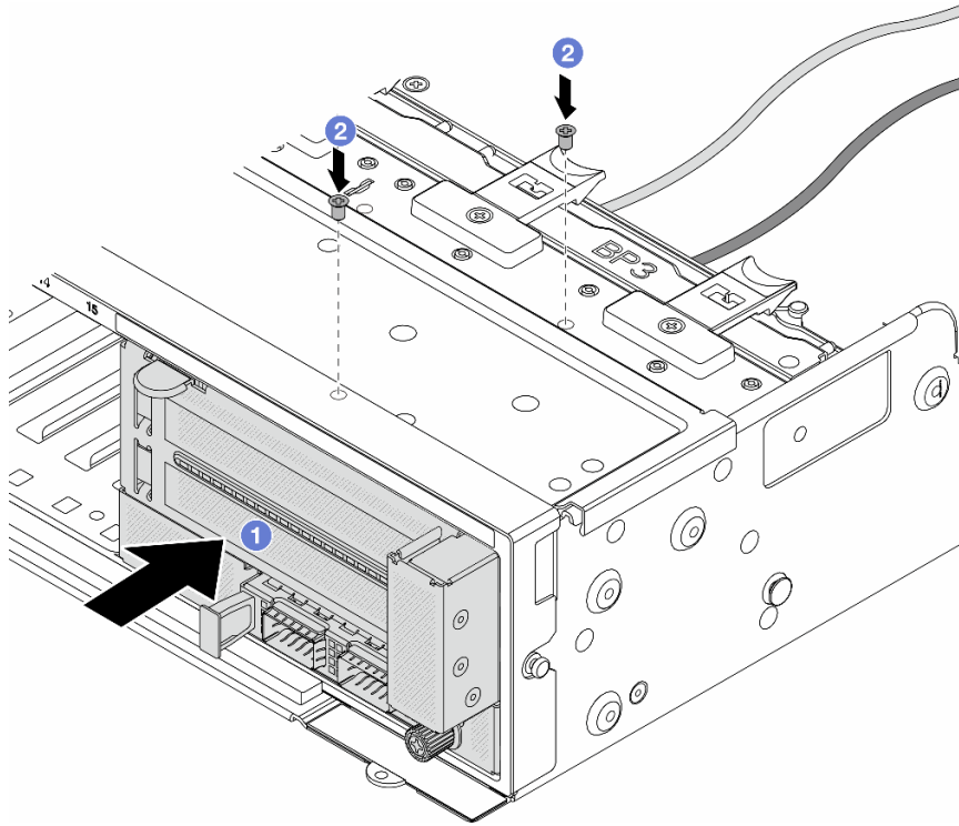
그림 44. 앞면 어댑터 어셈블리 설치
