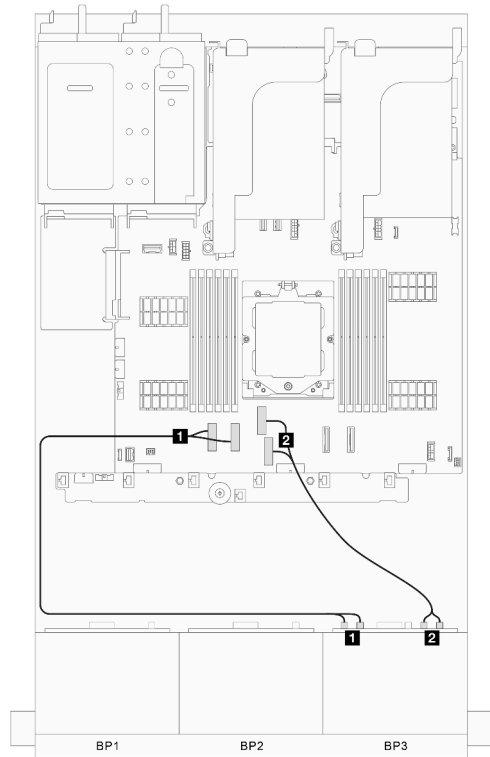
그림 334. 신호 케이블 배선 파트 2
