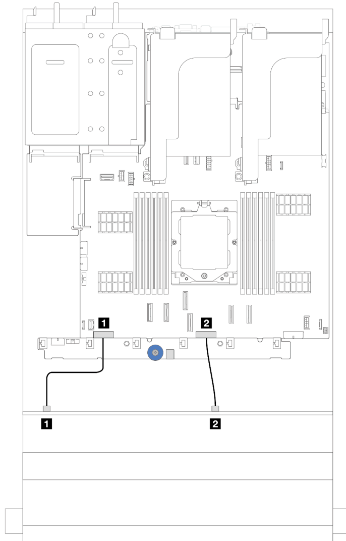
그림 373. 12 x 3.5" SAS/SATA 및 AnyBay 드라이브 백플레인의 전원 케이블 배선
