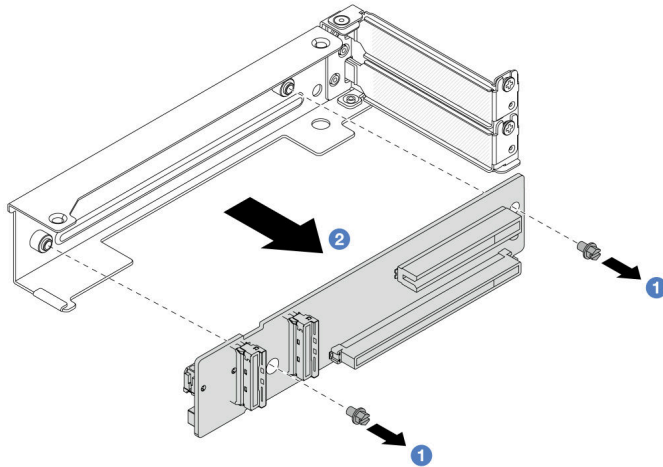
그림 139. 4LP 라이저 3/4 케이스에서 라이저 카드 제거
