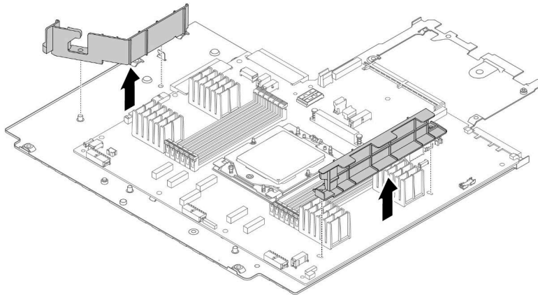
그림 412. 프로세서 보드에서 구성 요소 제거
