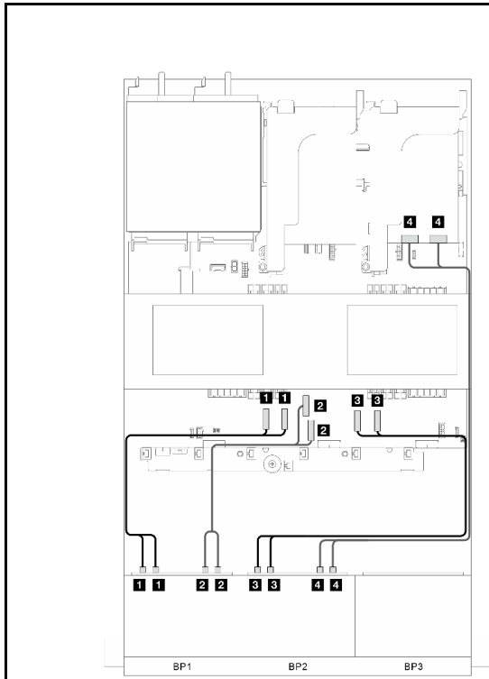
그림 366. 신호 케이블 배선 파트 1
