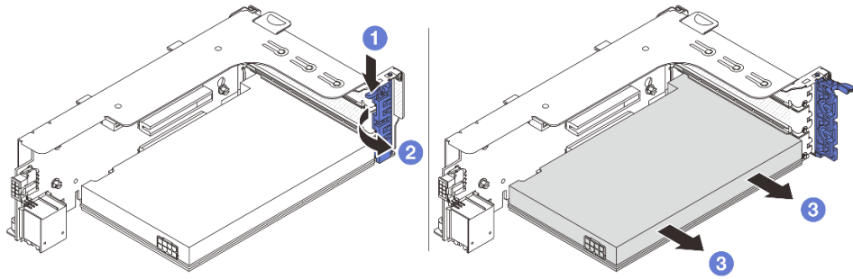
그림 134. 라이저 1 또는 2 어셈블리에서 PCIe 어댑터 제거
