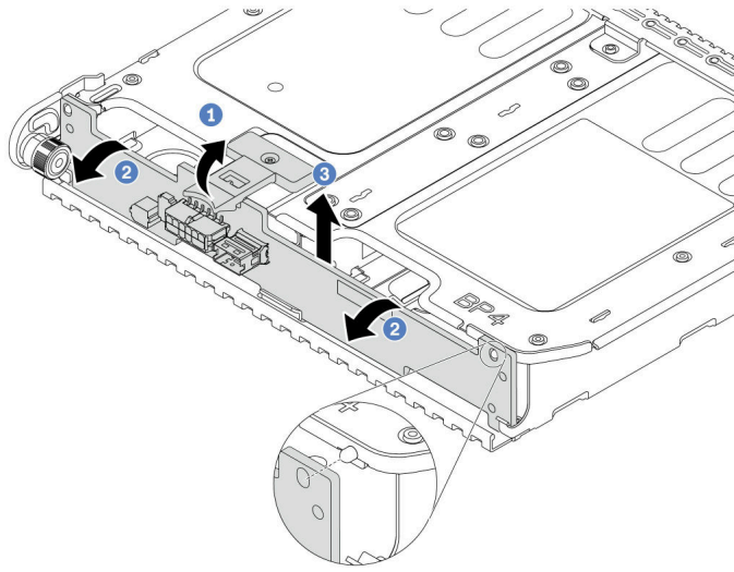
그림 222. 2 x 3.5" 뒷면 드라이브 백플레인 제거
