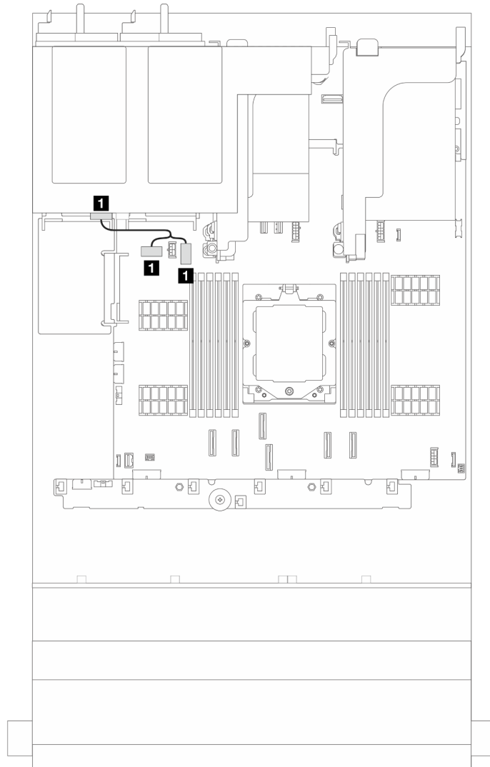
그림 375. 2 x 3.5" 및 4 x 2.5" 뒷면 드라이브 백플레인의 전원 케이블 배선
