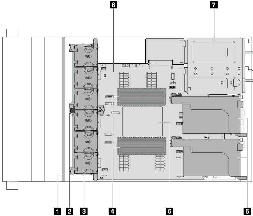
그림 9. 서버 평면도
