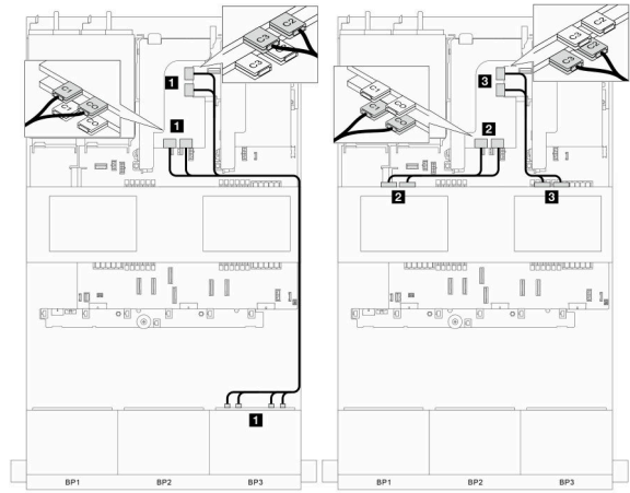
그림 367. 신호 케이블 배선 파트 2
