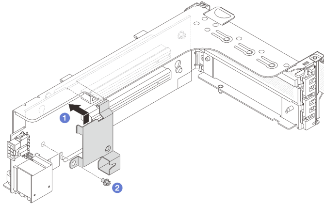
그림 209. 7mm 드라이브 케이지 고정 클립 설치
