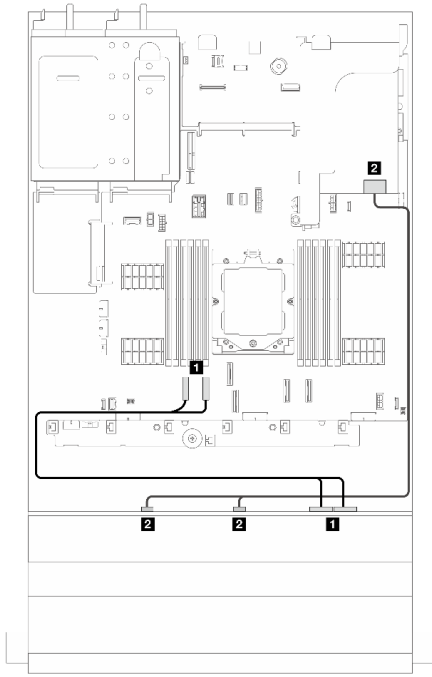
그림 382. 신호 케이블 배선
