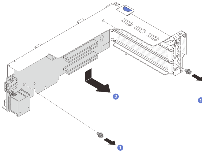
그림 137. 라이저 카드 1 제거(라이저 카드 2와 동일)
