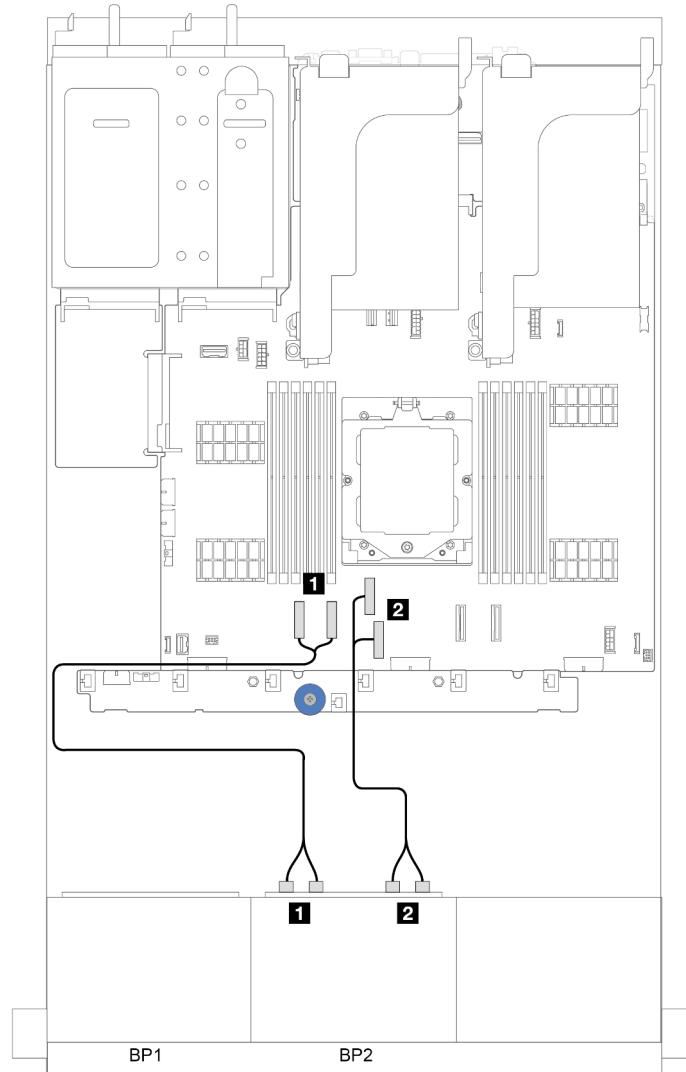
그림 319. 온보드 커넥터에 대한 NVMe 케이블 배선
