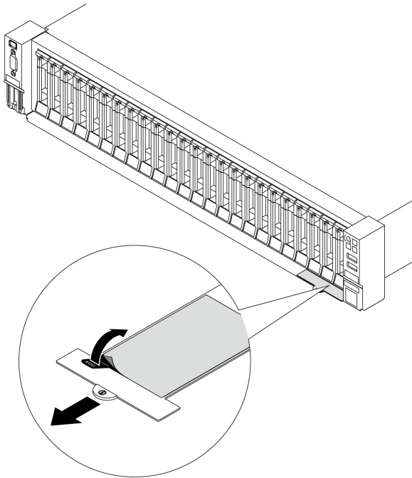
그림 15. 탈착식 정보 탭에 있는 Lenovo XClarity Controller 네트워크 액세스 레이블
