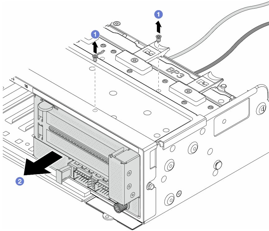
그림 47. 앞면 어댑터 어셈블리 제거
