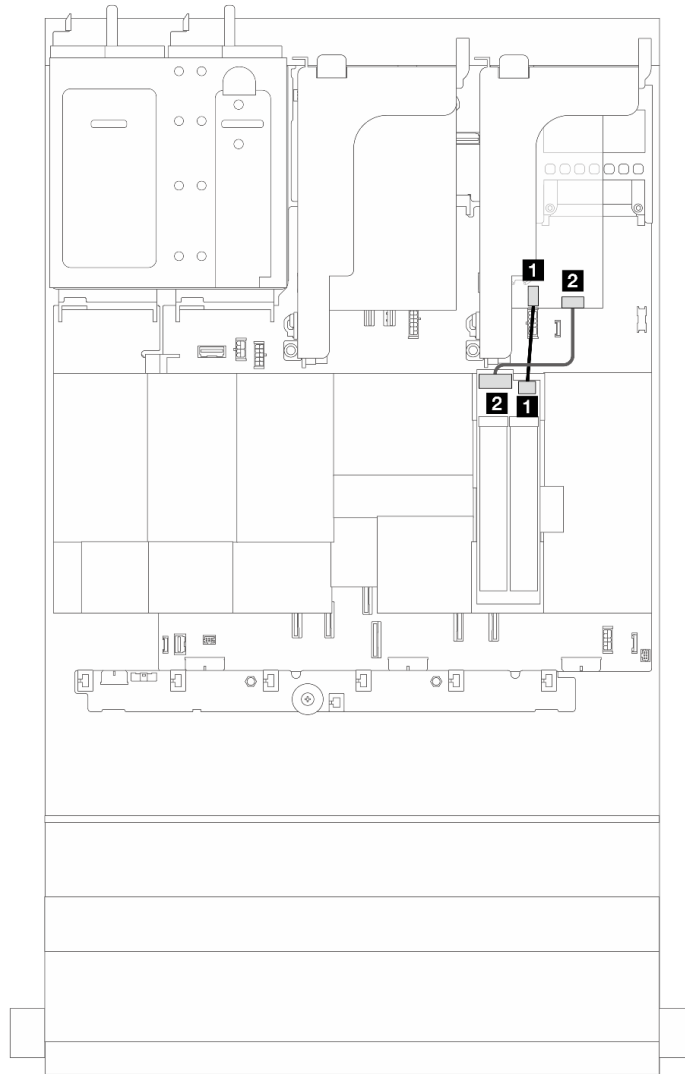
그림 284. M.2 드라이브 백플레인의 RAID 케이블 배선
