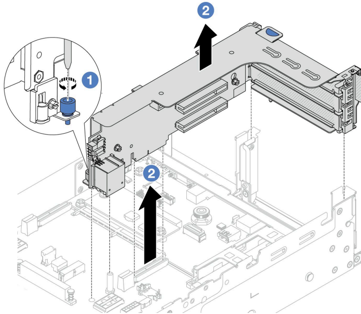
그림 130. 라이저 1 어셈블리 제거
