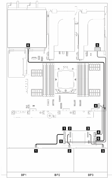
그림 346. 신호 케이블 배선 파트 1
