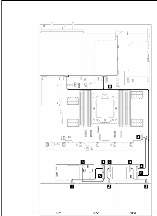
그림 350. 신호 케이블 배선 파트 1
