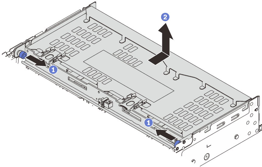
그림 225. 4 x 3.5" 뒷면 드라이브 케이스 제거
