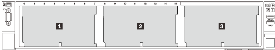
그림 69. 드라이브 백플레인 numbering
