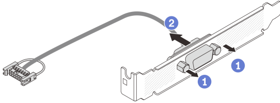
그림 249. 직렬 포트 모듈 분해
