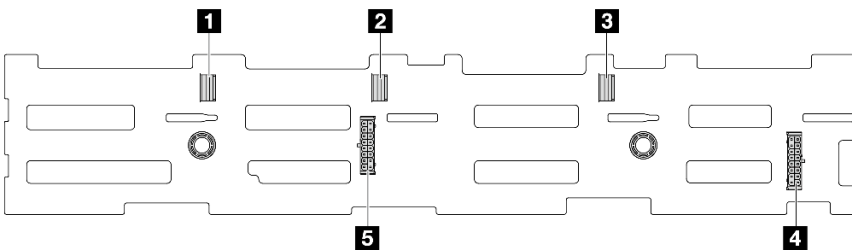
그림 260. 12 x 3.5" SAS/SATA 백플레인 커넥터
