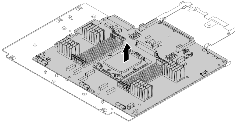
그림 413. 지지 판금에서 프로세서 보드 분리
