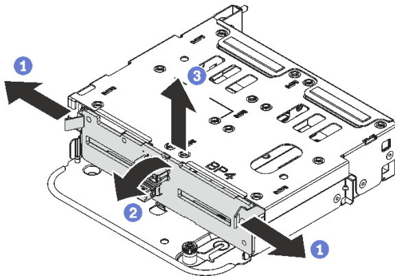
그림 214. 4 x 2.5" 뒷면 드라이브 백플레인 제거
