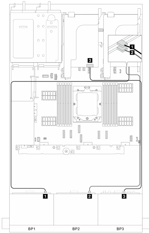
그림 331. 신호 케이블 배선 파트 1
