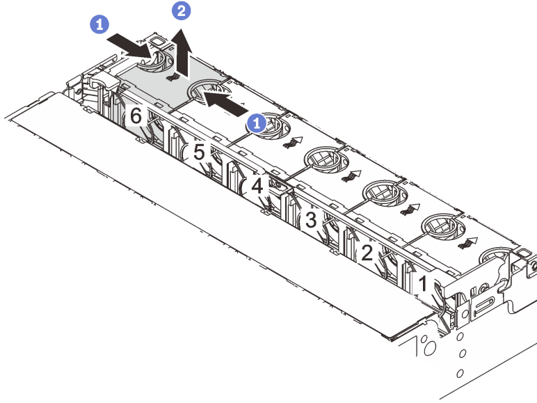
그림 242. 시스템 팬 제거
