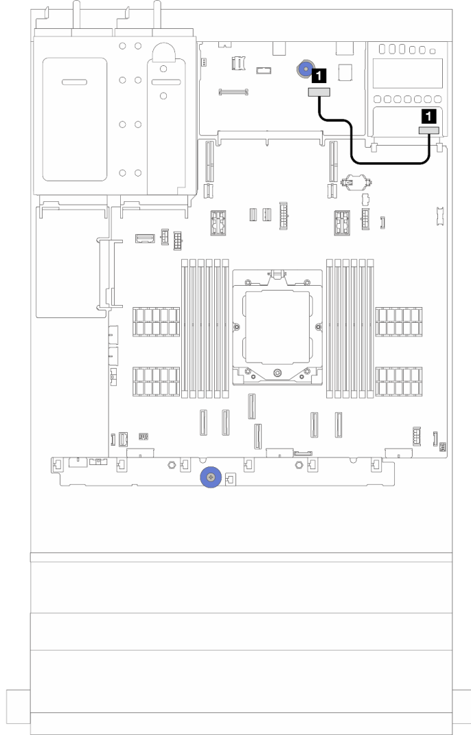
그림 289. 관리 NIC 어댑터의 케이블 배선
