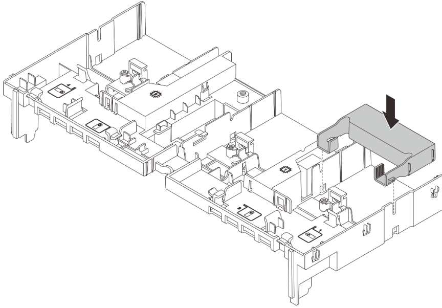
그림 89. 추가 공기 조절 장치 설치
