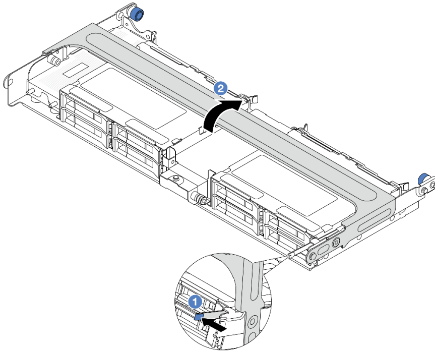
그림 193. 중간 드라이브 케이지의 손잡이 닫기
