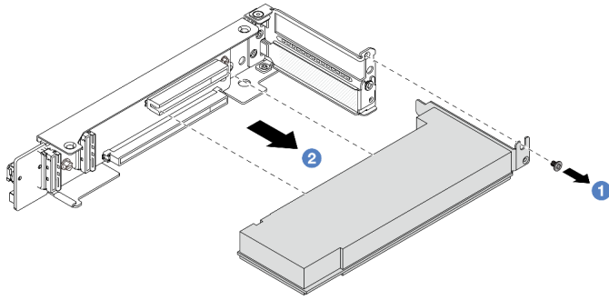
그림 136. 4LP 라이저 3/4 어셈블리에서 PCIe 어댑터 제거
