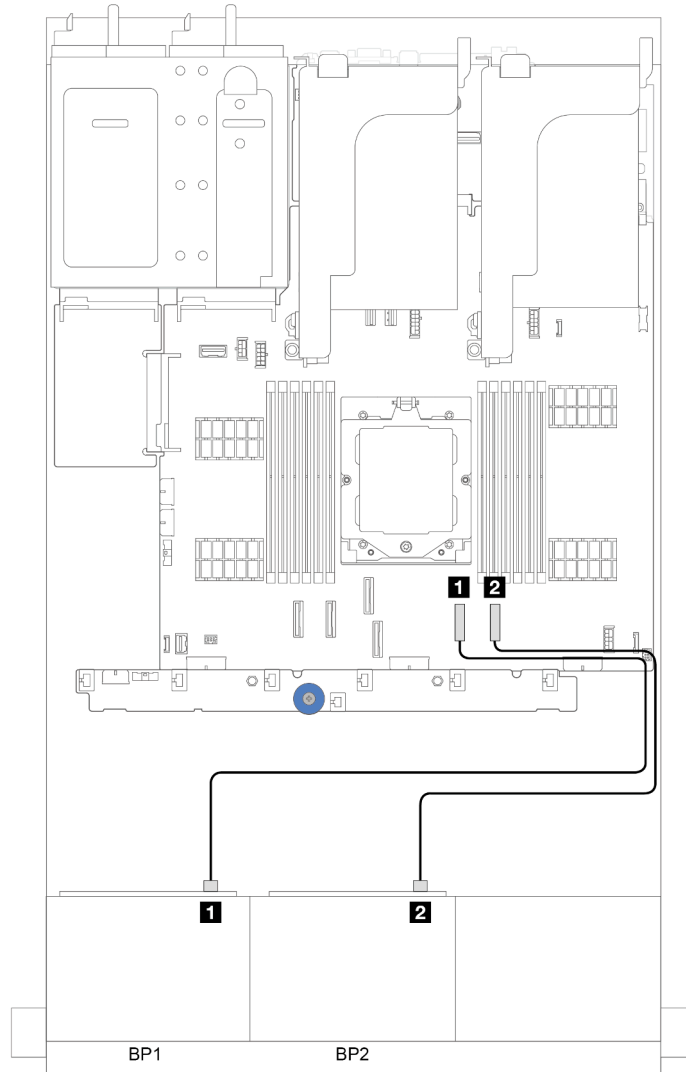
그림 315. 온보드 SATA 커넥터에 대한 SAS/SATA 케이블 배선
