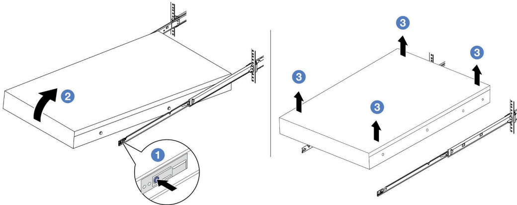
그림 20. 랙에서 서버 제거
