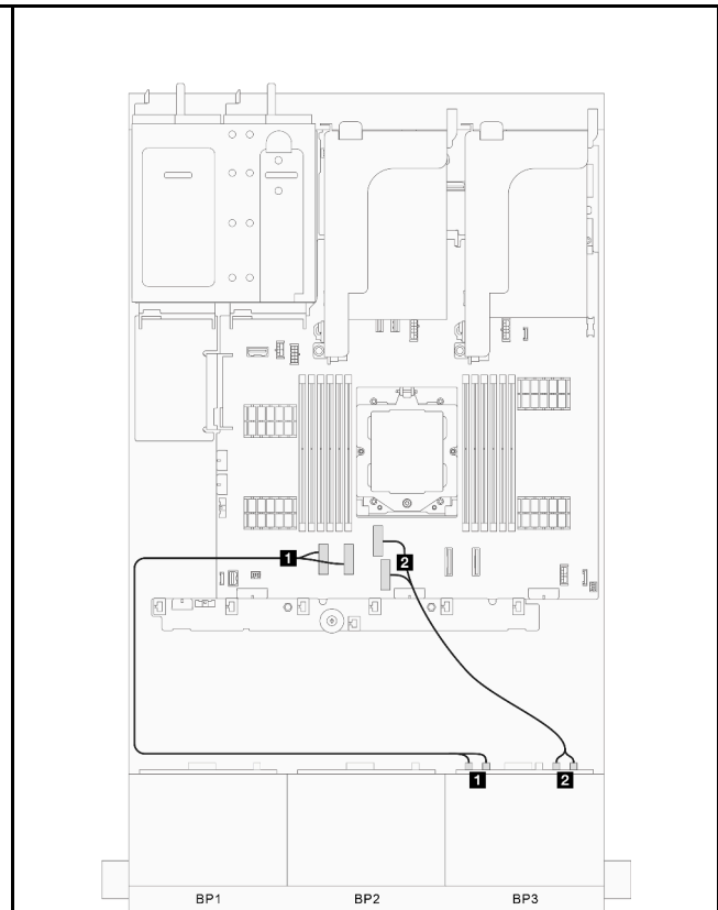
그림 328. 신호 케이블 배선 파트 2
