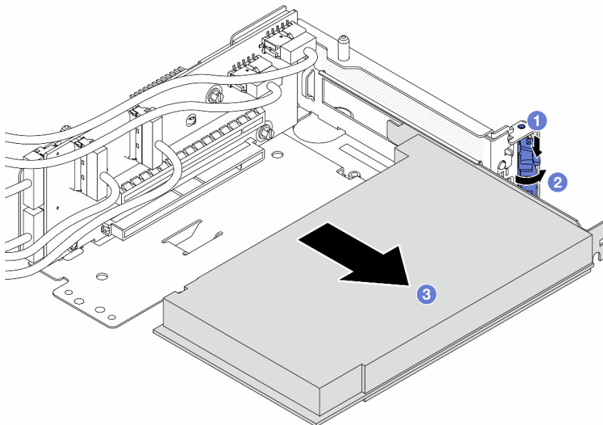
그림 35. 라이저 5 케이지에서 PCIe 어댑터 제거
