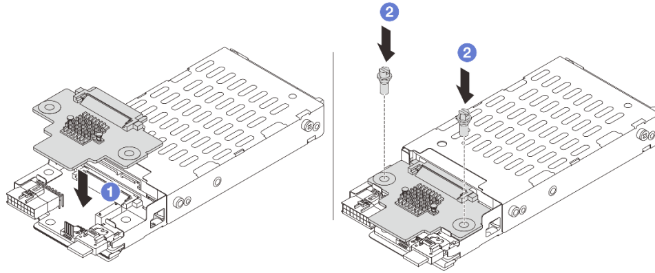
그림 208. 7mm 드라이브 백플레인 설치(상단)
