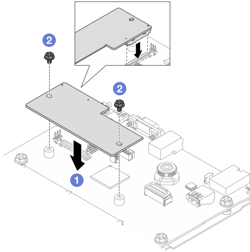
그림 237. 펌웨어 및 RoT 보안 모듈 설치
