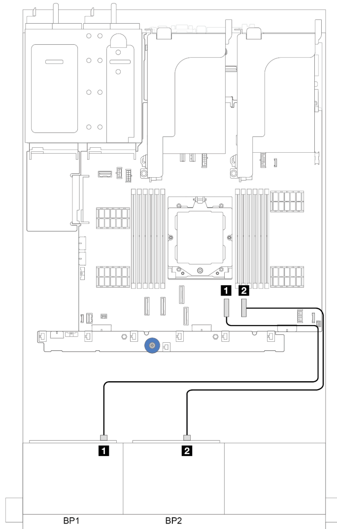
그림 318. 온보드 커넥터에 대한 SAS/SATA 케이블 배선
