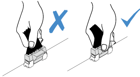
그림 86. 시스템 보드 어셈블리에서 케이블 분리
