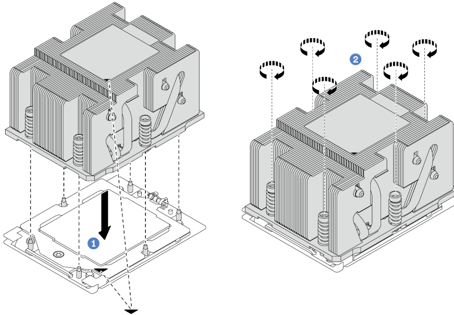
그림 166. 표준 방열판 설치
