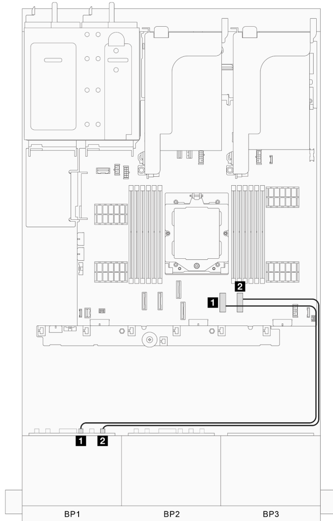
그림 312. 온보드 커넥터(라이저 3 지원)
