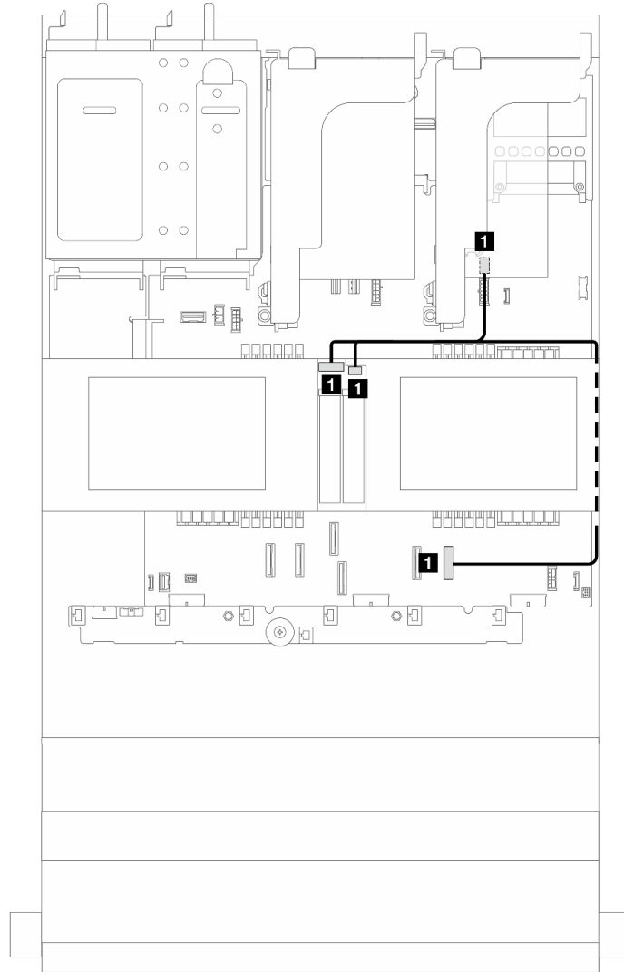
그림 281. M.2 드라이브 백플레인의 SATA 케이블 배선
