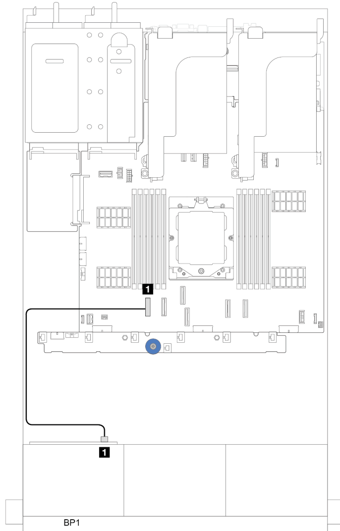
그림 314. 프로세서 1개가 설치된 경우 케이블 배선
