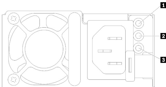
Рис. 16. Светодиодные индикаторы блока питания
