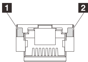
Рис. 15. Порт управления системой ХСС Светодиодные индикаторы
