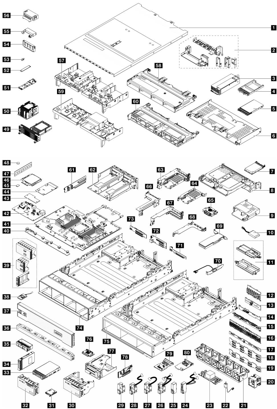
Рис. 19. Компоненты сервера
