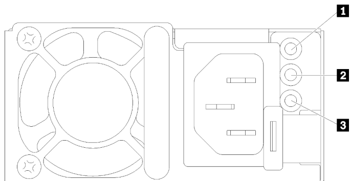
รูปภาพ 16. ไฟ LED แหล่งจ่ายไฟ
