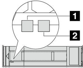
รูปภาพ 13. ไฟ LED ของไดรฟ์
