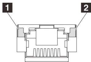
รูปภาพ 15. พอร์ตการจัดการระบบ XCC ไฟ LED
