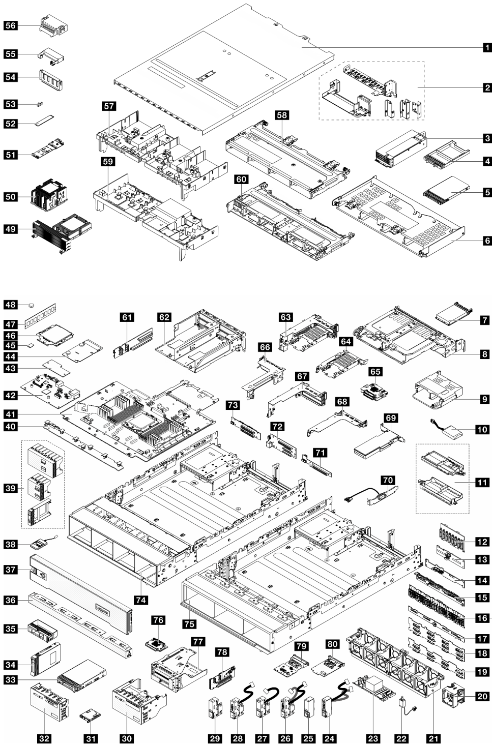
รูปภาพ 19. ส่วนประกอบเซิร์ฟเวอร์
