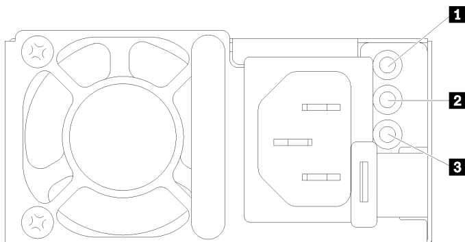
圖例 16. 電源供應器 LED
