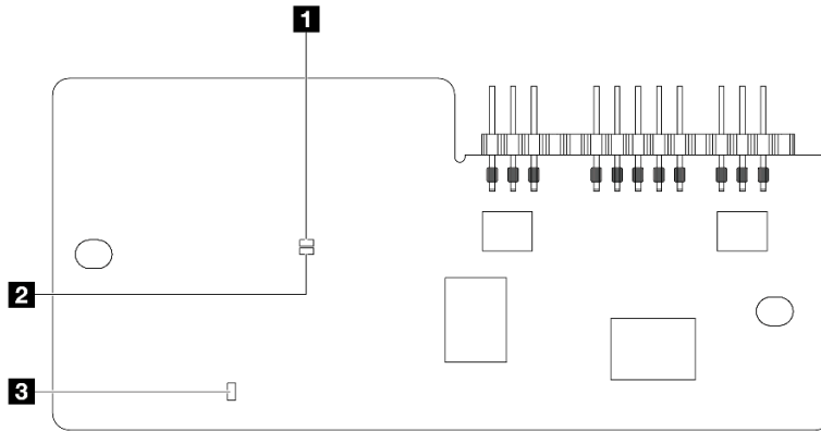
圖例 18. 韌體和 RoT 安全模組上的 LED
