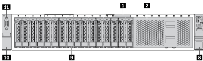
Figura 2. Modelos de servidor con dieciséis bahías de unidad de 2,5 pulgadas
