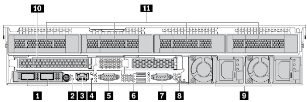
그림 8. PCIe 슬롯 2개 및 뒷면 3.5인치 드라이브 베이 4개 지원 서버 모델
