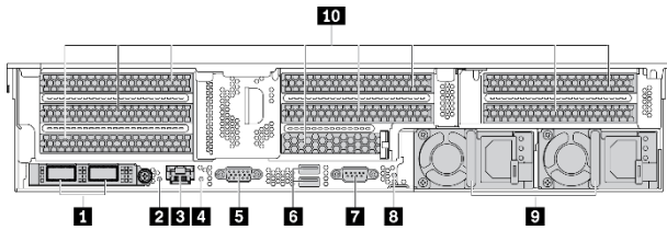
그림 6. 8개의 PCIe 슬롯이 있는 서버 모델
