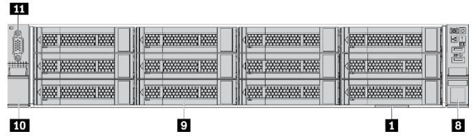
그림 5. 12개의 3.5인치 드라이브 베이 지원 서버 모델
