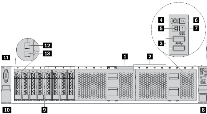
그림 1. 8개의 2.5인치 드라이브 베이 지원 서버 모델
