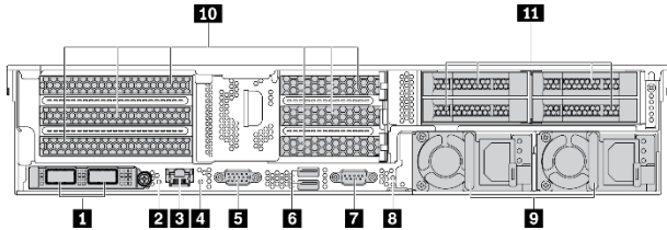
그림 7. PCIe 슬롯 6개 및 뒷면 2.5인치 드라이브 베이 4개 지원 서버 모델
