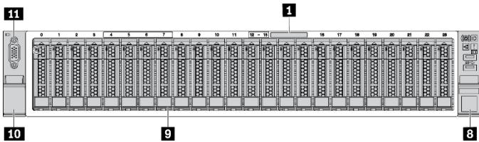
그림 3. 24개의 2.5인치 드라이브 베이 지원 서버 모델
