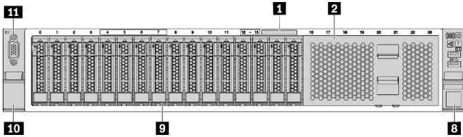
그림 2. 16개의 2.5인치 드라이브 베이 지원 서버 모델
