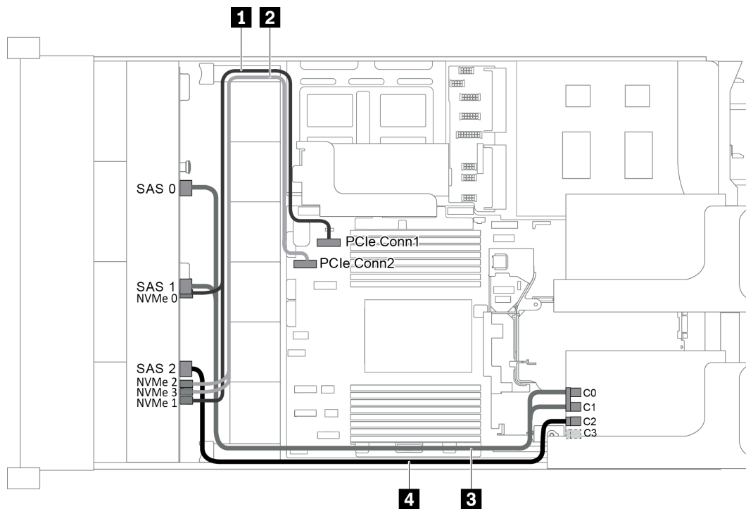
圖例 54. 配置為一個 12 x 3.5 吋 AnyBay 前方背板和一張 16i RAID/HBA 配接卡的纜線佈線
