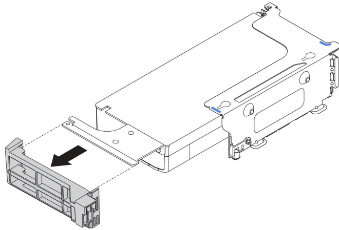
圖例 219. 卸下雙寬 GPU 配接卡適用的 GPU 空氣擋板附加元件
