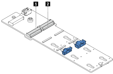
圖例 147. M.2 硬碟插槽
