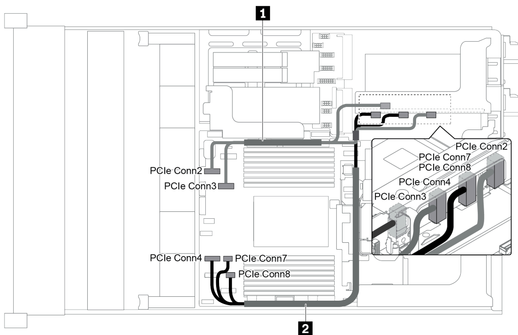
圖例 35. 擴充卡 3 (x16/x16 PCIe) 的纜線佈線
