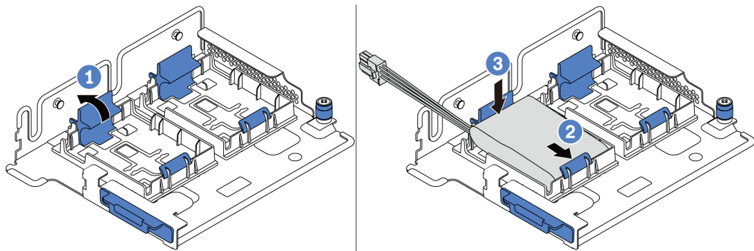
圖例 136. 超級電容器模組安裝
