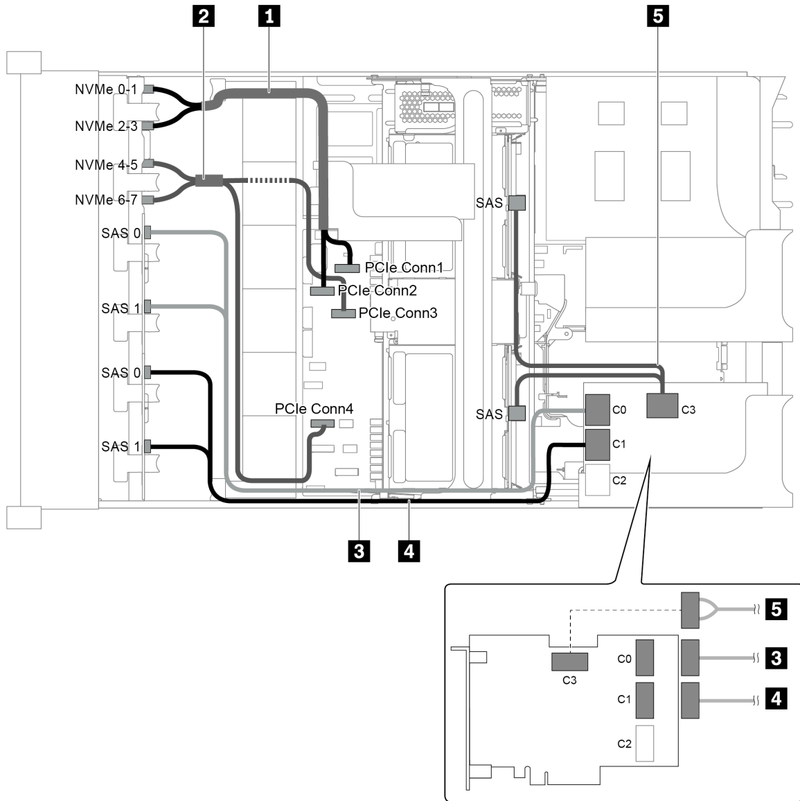
圖例 96. 配置為三個前方背板 (8 NVMe + 2 x 8 SAS/SATA)、一個中間框架和一張 32i RAID 配接卡的纜線佈線
