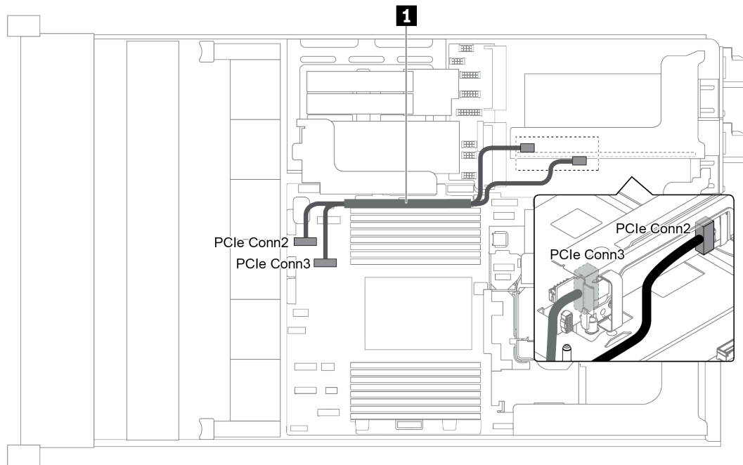
圖例 34. 擴充卡 3 (x8/x8 PCIe) 的纜線佈線
