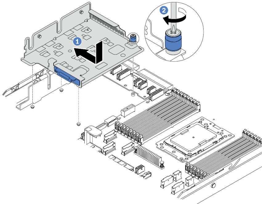
圖例 134. 支撐托架安裝
