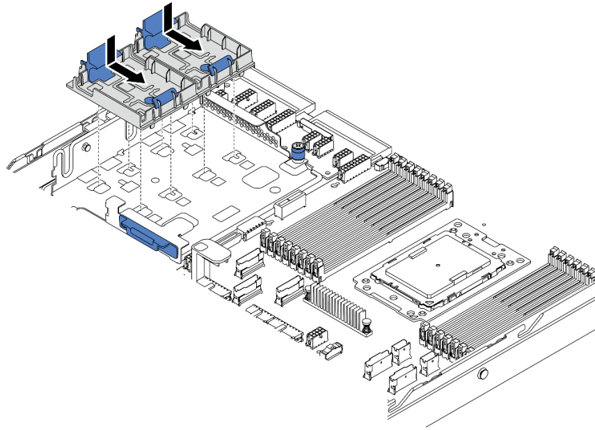
圖例 135. 超級電容器固定器安裝
