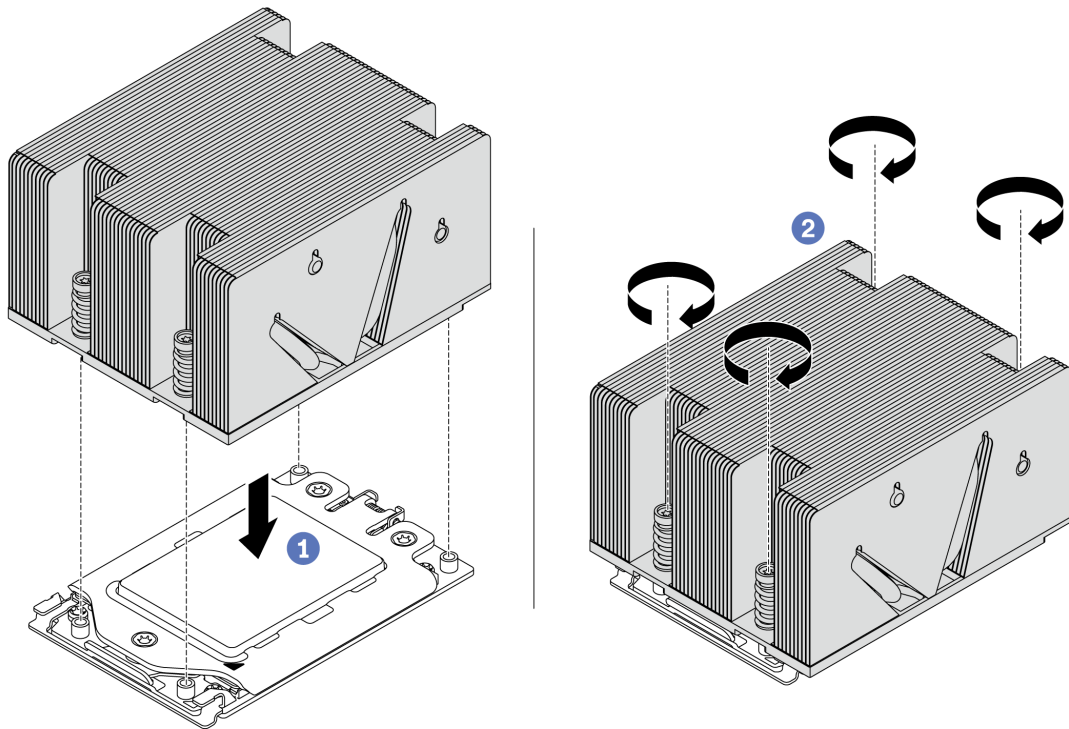
圖例 246. 安裝散熱槽
