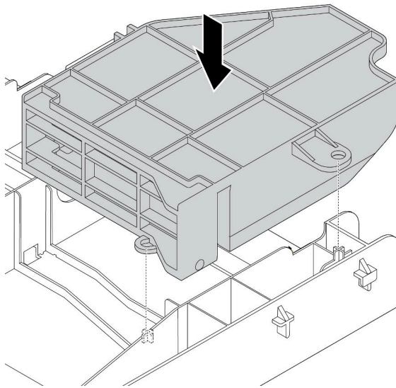
圖例 222. 安裝單倍寬 GPU 配接卡適用的 GPU 空氣擋板附加元件
