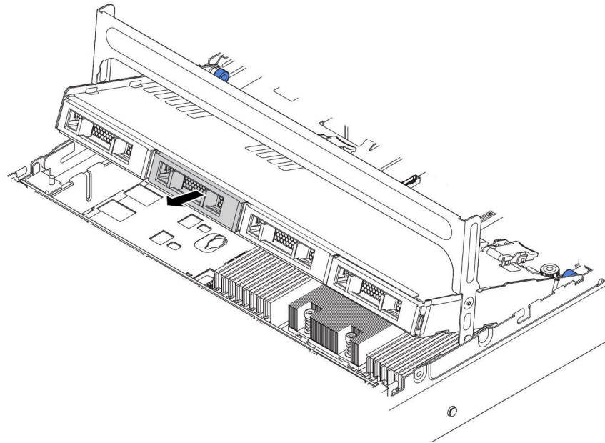
圖例 181. 從中間 3.5 吋框架卸下硬碟
