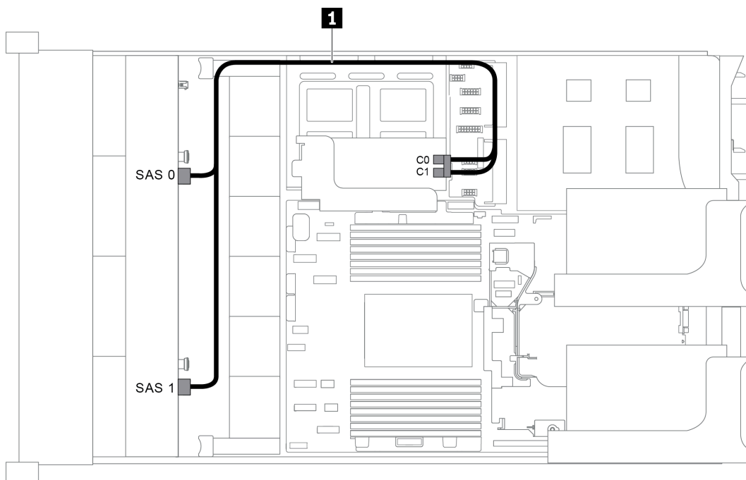
圖例 44. 配置為一個 8 x 3.5 吋 SAS/SATA 前方背板和一張 8i RAID/HBA 配接卡的纜線佈線
