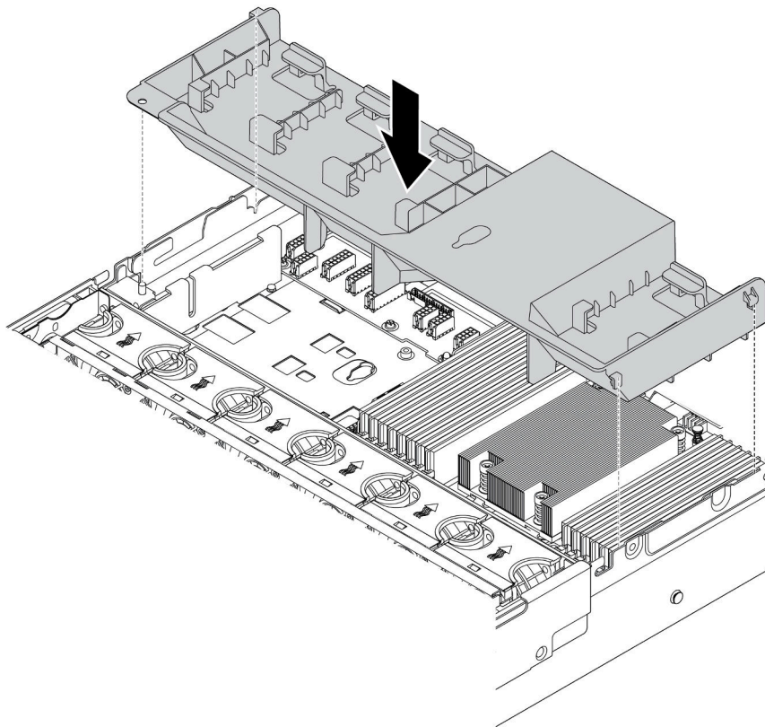
圖例 126. 安裝標準空氣擋板
