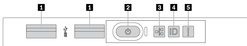
圖例 11. 配備八個 3.5 吋機槽之伺服器型號的正面 I/O 組件
