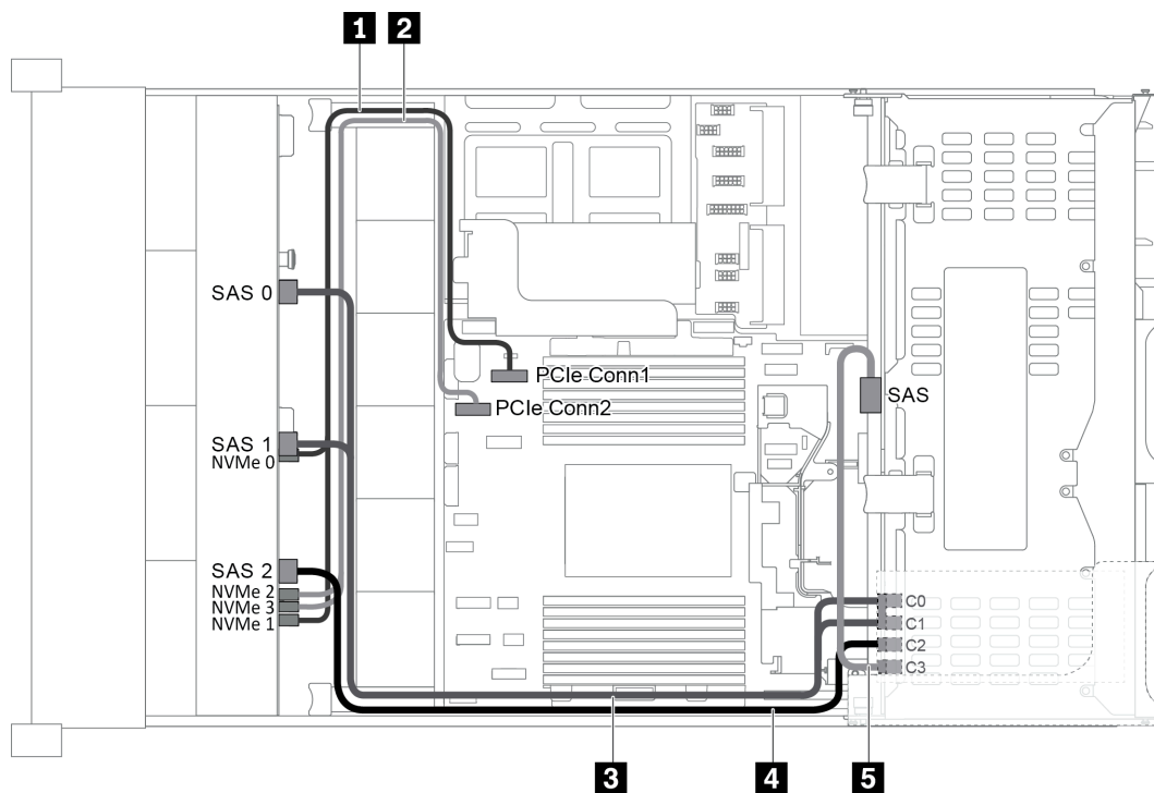
圖例 55. 配置為一個 12 x 3.5 吋 AnyBay 前方背板、一個後方框架和一張 16i RAID/HBA 配接卡的纜線佈線
