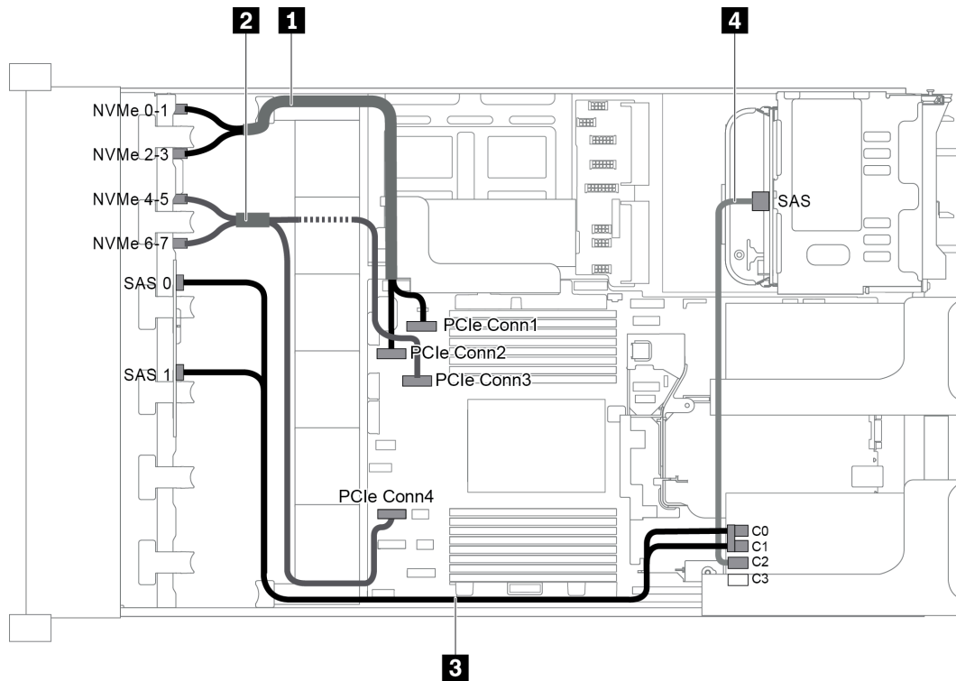
圖例 71. 配置為兩個前方背板 (8 NVMe + 8 SAS/SATA)、一個背面框架和一張 16i RAID/HBA 配接卡的纜線佈線
