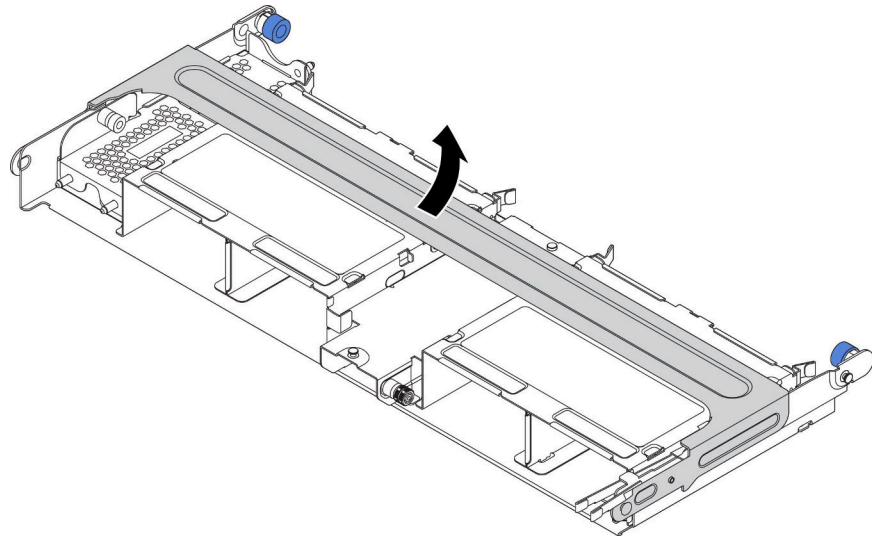
圖例 129. 打開中間框架的把手
