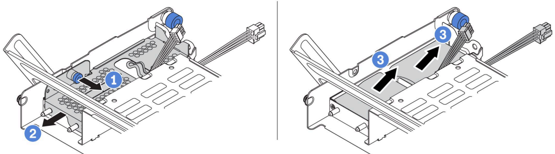
圖例 130. 卸下超級電容器模組
