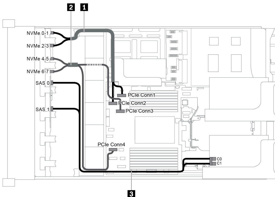
圖例 70. 配置為兩個前方背板 (8 NVMe + 8 SAS/SATA) 和一張 8i RAID/HBA 配接卡的纜線佈線
