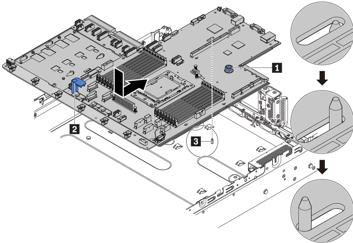
圖例 253. 安裝主機板
