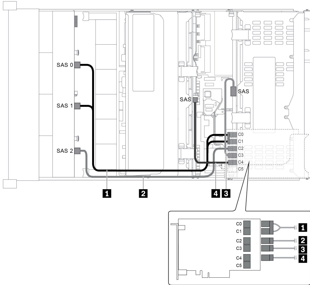
圖例 50. 配置為一個 12 x 3.5 吋 SAS/SATA 前方背板、一個背面框架、一個中間框架和一張 24i RAID 配接卡的纜線佈線
