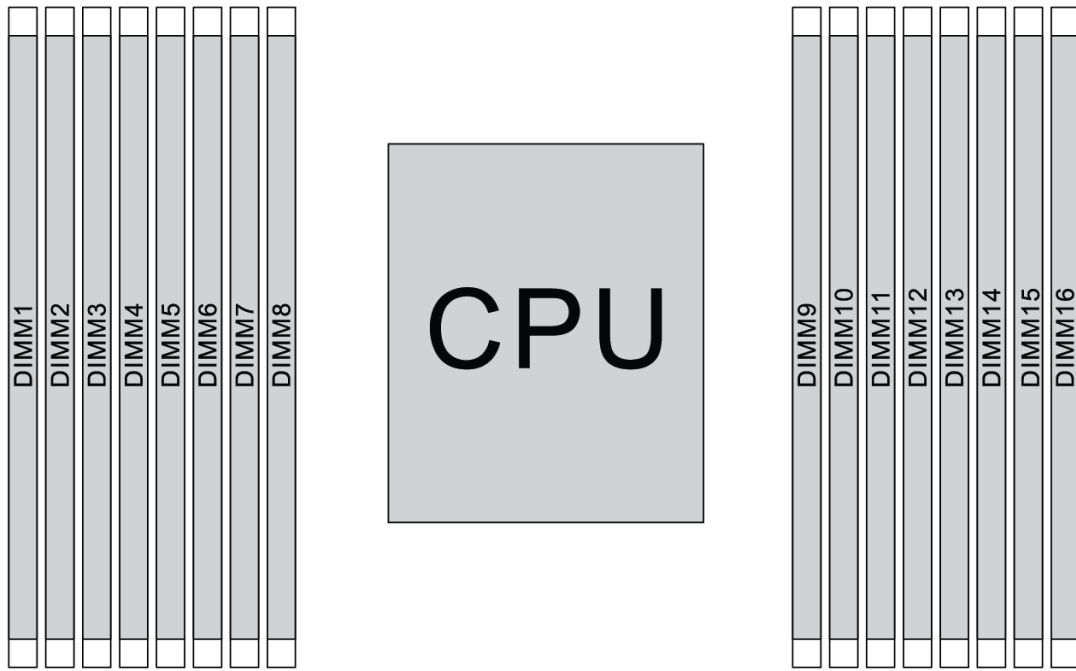
圖例 109. DIMM 位置
