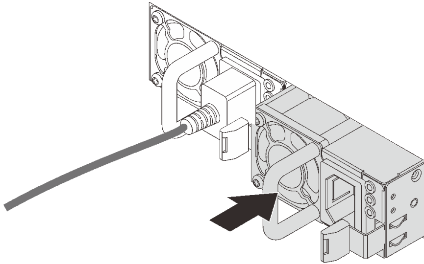
圖例 241. 安裝熱抽換電源供應器
