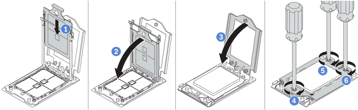
圖例 244. 安裝處理器
