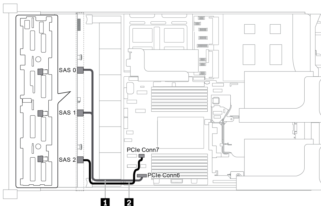
圖例 45. 配置為一個 12 x 3.5 吋 SAS/SATA 前方背板的纜線佈線
