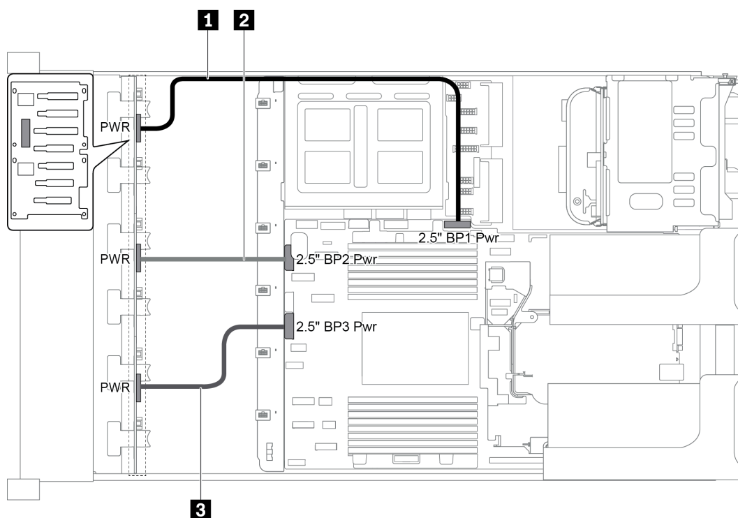
圖例 37. 前方 2.5 吋硬碟背板的電源佈線
