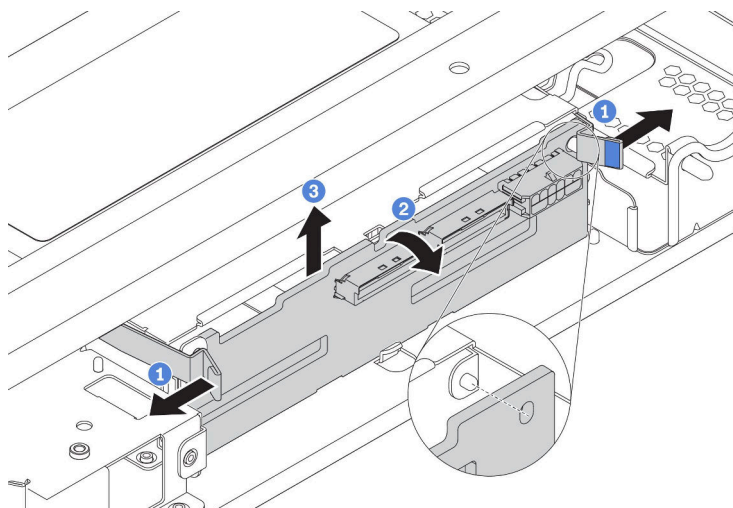
圖例 169. 卸下中間或後方 2.5 吋硬碟背板
