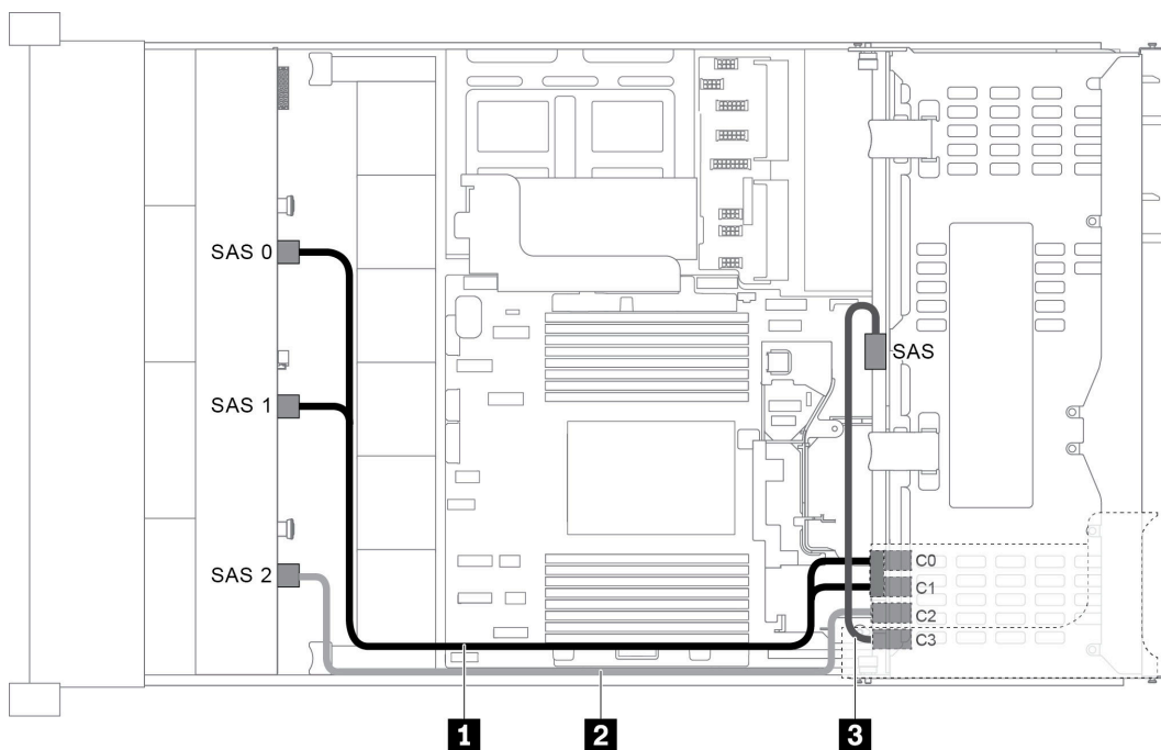
圖例 48. 配置為一個 12 x 3.5 吋 SAS/SATA 前方背板、一個背面框架和一張 16i RAID/HBA 配接卡的纜線佈線
