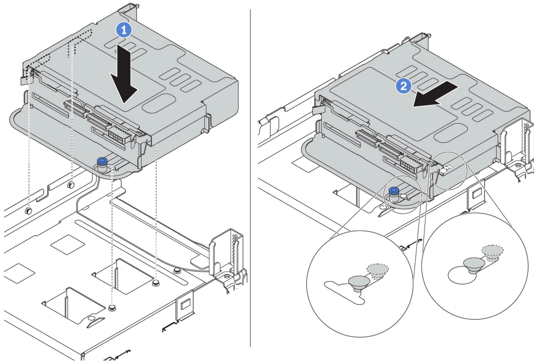
圖例 231. 安裝背面 2.5 吋框架
