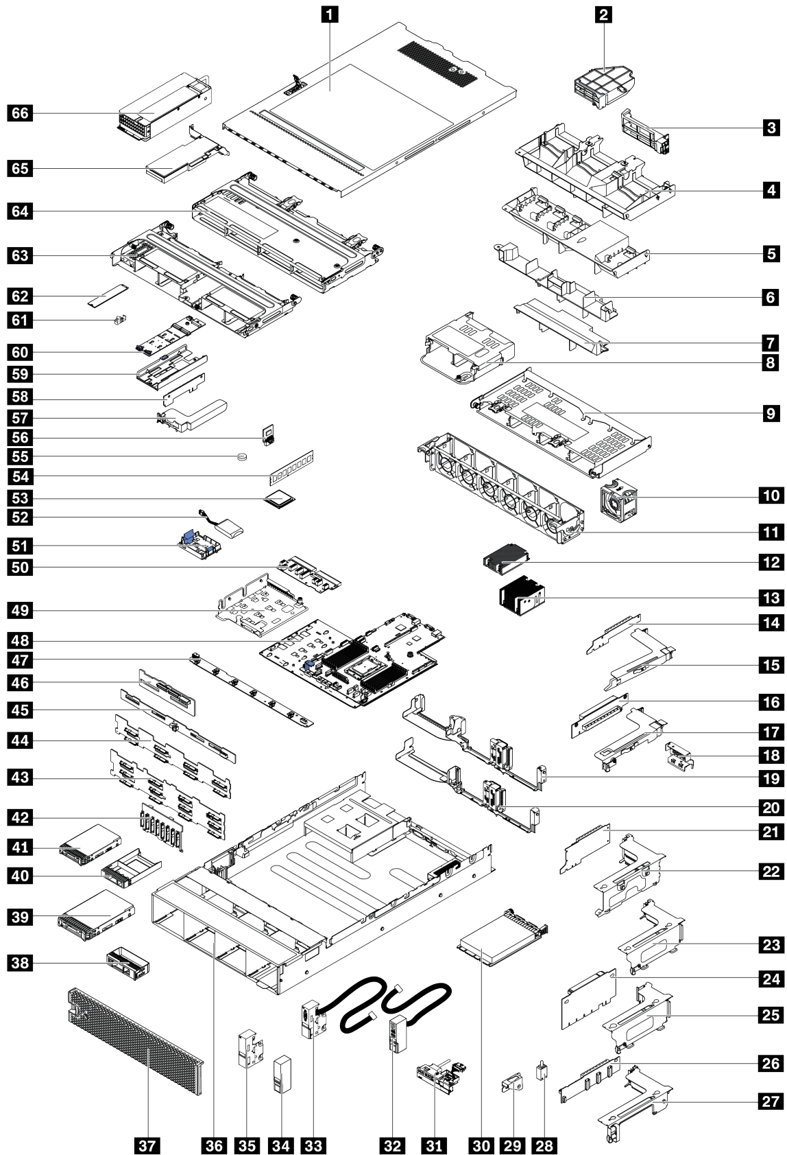
圖例 22. 伺服器元件
