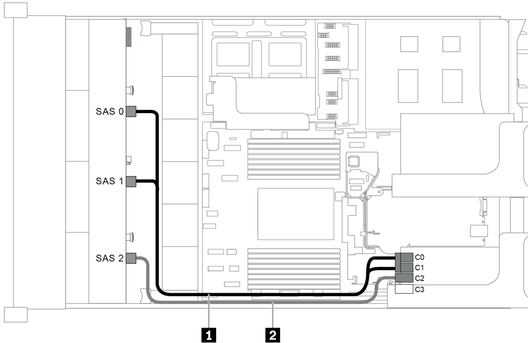
圖例 46. 配置為一個 12 x 3.5 吋 SAS/SATA 前方背板和一張 16i RAID/HBA 配接卡的纜線佈線
