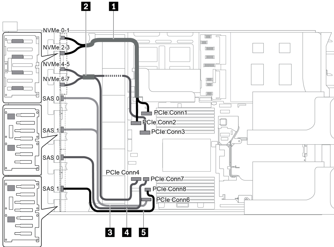
圖例 86. 配置為三個前方背板 (8 NVMe + 2 x 8 SAS/SATA) 的纜線佈線
