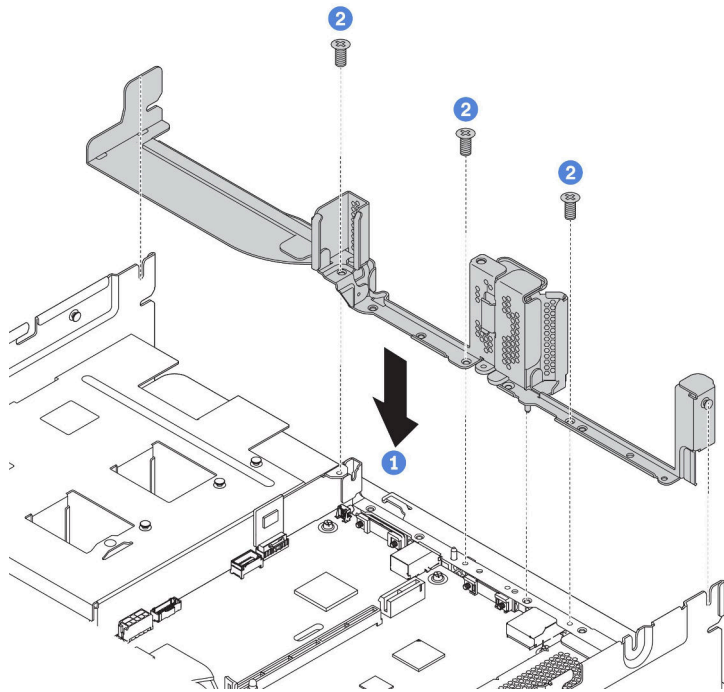
圖例 230. 安裝背面 2.5 吋框架的後壁托架
