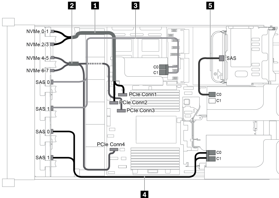
圖例 91. 配置為三個前方背板 (8 NVMe + 2 x 8 SAS/SATA)、一個後方框架和三張 8i RAID/HBA 配接卡的纜線佈線
