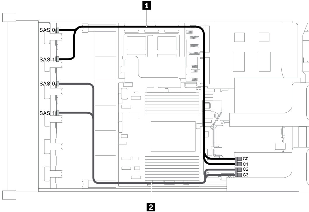
圖例 63. 配置為兩個 8 x 2.5 吋 SAS/SATA 前方背板和一張 16i RAID/HBA 配接卡的纜線佈線
