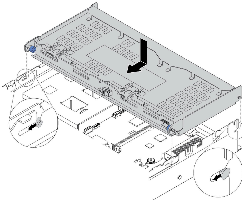
圖例 234. 安裝背面 3.5 吋框架
