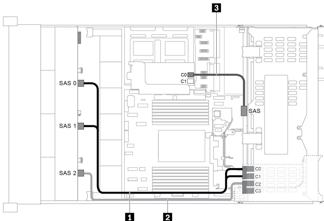
圖例 49. 配置為一個 12 x 3.5 吋 SAS/SATA 前方背板、一個框架和兩張 RAID/HBA 配接卡的纜線佈線 (8i+16i)
