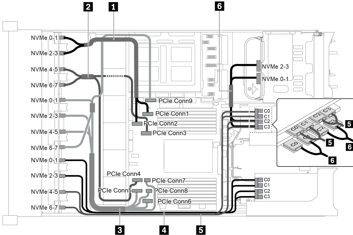
圖例 100. 配置為三個 8 x 2.5 吋 NVMe 前方背板、一個背面框架 (NVMe) 和三張 810-4P 或 1610-4P NVMe 交換器卡的纜線佈線
