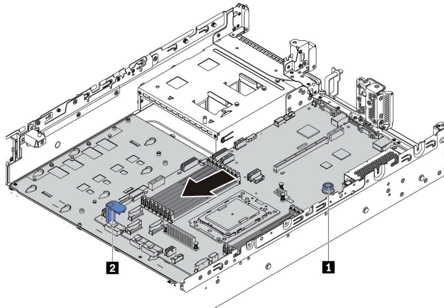
圖例 251. 卸下主機板 (1)
