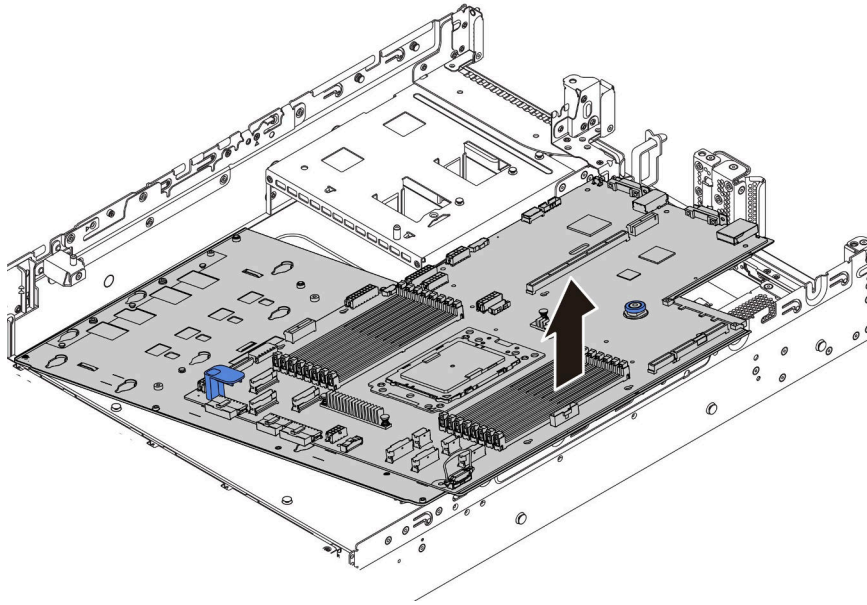
圖例 252. 卸下主機板 (2)
