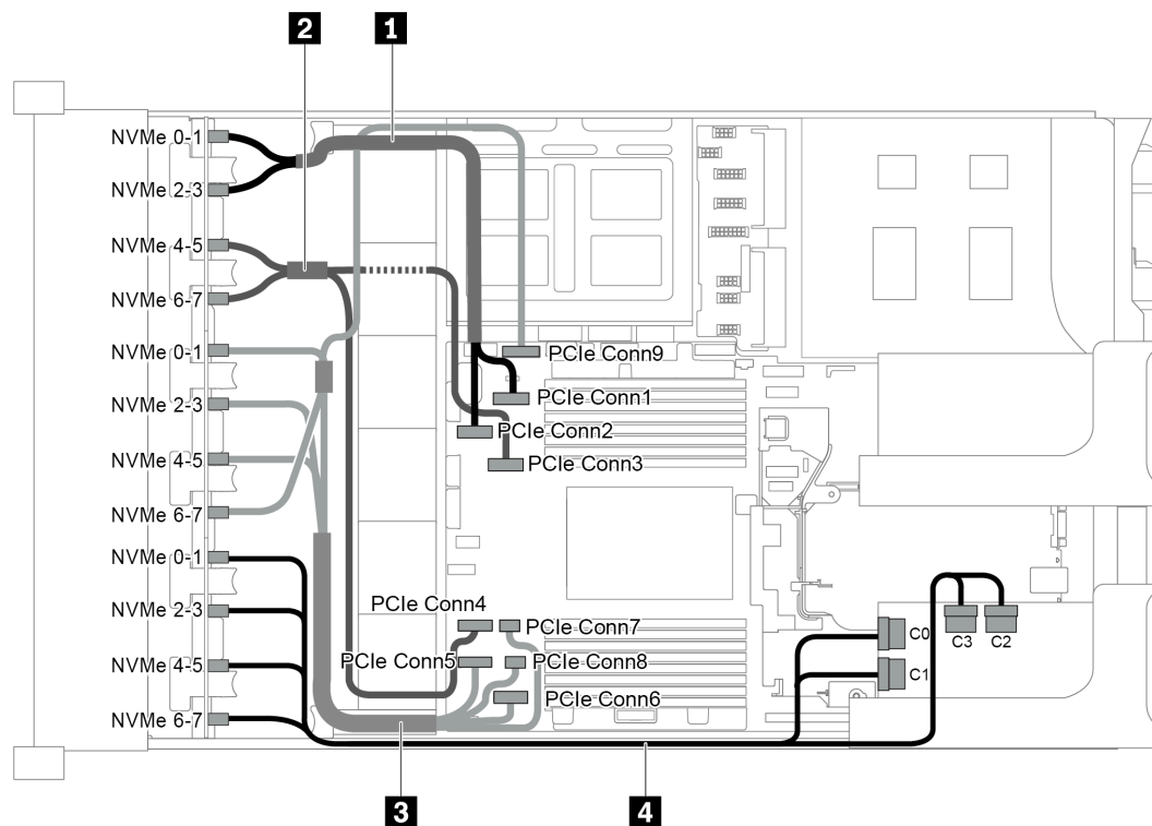
圖例 98. 配置為三個 8 x 2.5 吋 NVMe 前方背板和一張 1611-8P NVMe 交換器卡的纜線佈線
