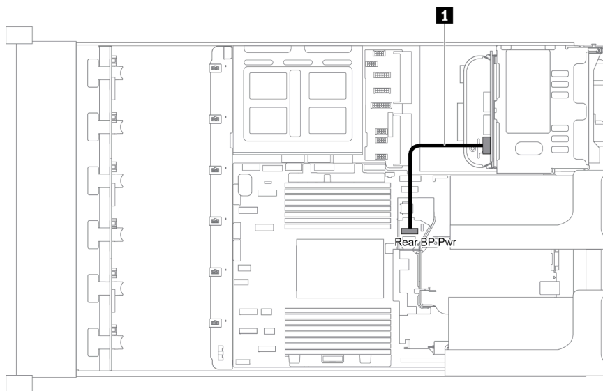
圖例 41. 後方 2.5 吋硬碟背板的電源佈線
