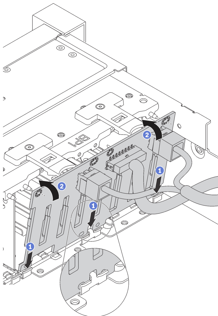
圖例 166. 2.5 吋硬碟背板安裝
