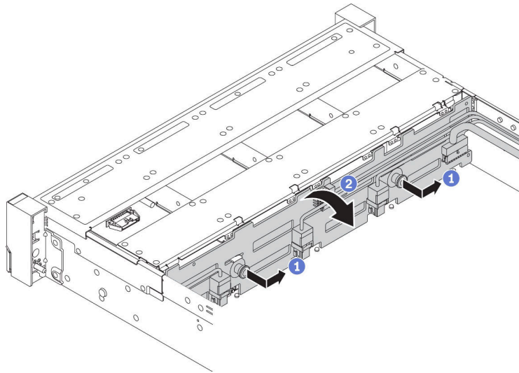
圖例 167. 卸下 3.5 吋硬碟背板
