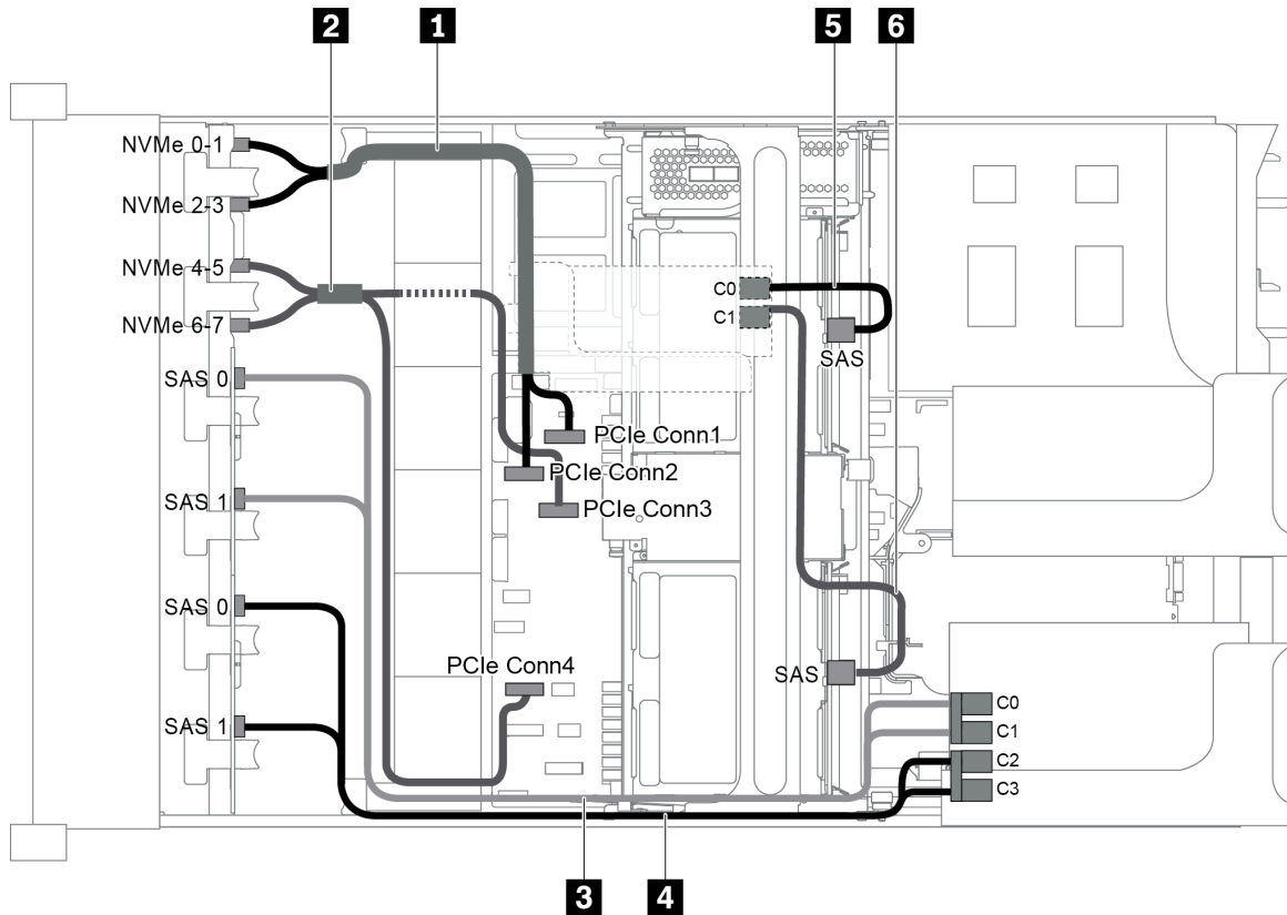
圖例 93. 配置為三個前方背板 (8 NVMe + 2 x 8 SAS/SATA)、一個中間框架和兩張 RAID/HBA 配接卡 (8i+16i) 的纜線佈線
