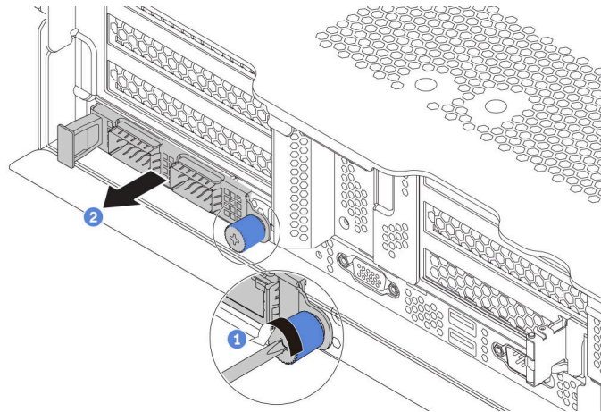
圖例 225. 卸下 OCP 3.0 乙太網路配接卡
