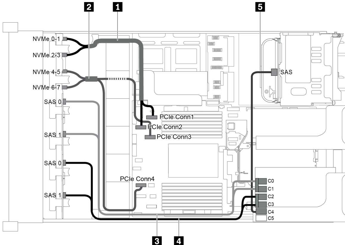
圖例 89. 配置為三個前方背板 (8 NVMe + 2 x 8 SAS/SATA)、一個背面框架和一張 24i RAID 配接卡的纜線佈線
