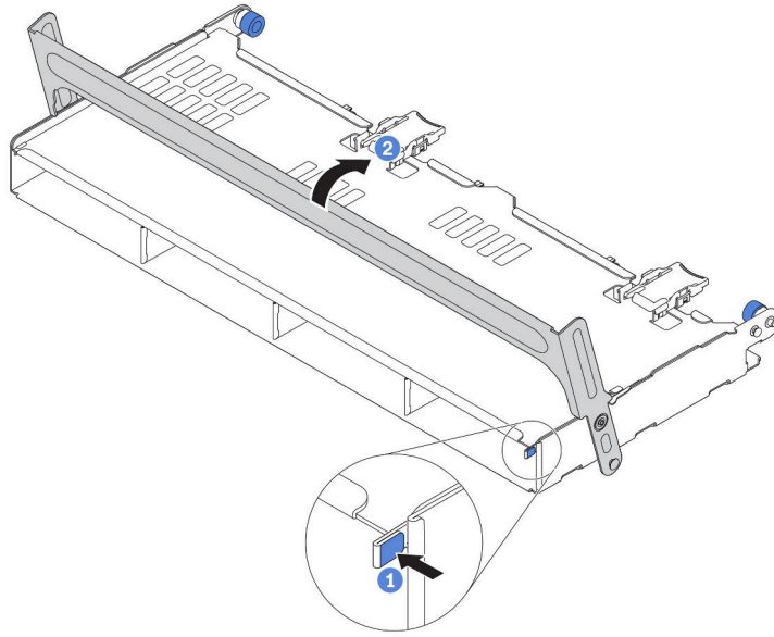
圖例 183. 合上中間 3.5 吋框架的把手
