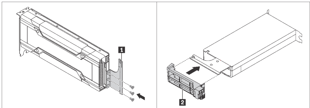
圖例 221. 安裝雙寬 GPU 配接卡適用的 GPU 空氣擋板附加元件
