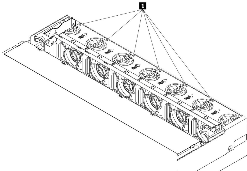
圖例 151. 從系統風扇頂端檢視風扇錯誤 LED
