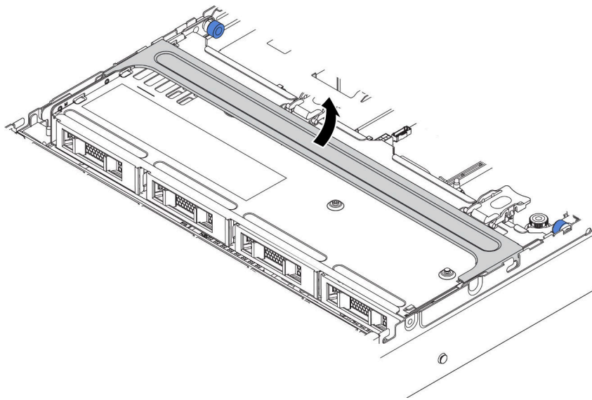
圖例 180. 打開框架把手
