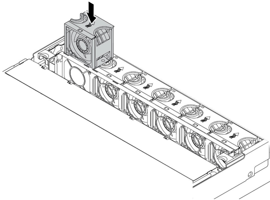
圖例 153. 安裝系統風扇
