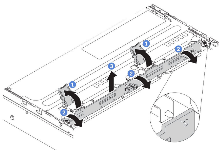
圖例 171. 卸下中間或後方 3.5 吋硬碟背板
