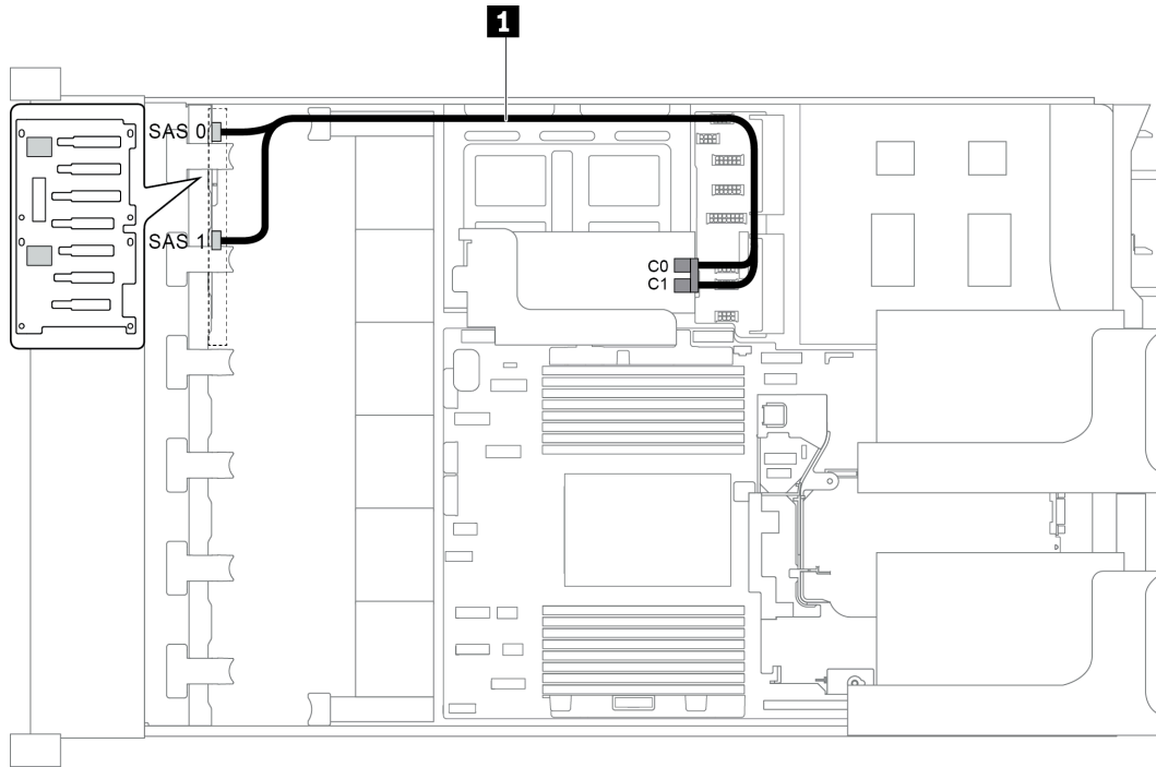
圖例 60. 配置為一個 8 x 2.5 吋 SAS/SATA 前方背板和一張 8i RAID/HBA 配接卡的纜線佈線
