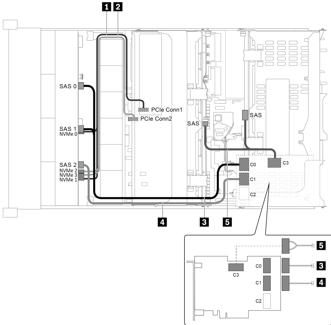
圖例 59. 配置為一個 12 x 3.5 吋 AnyBay 前方背板、一個後方框架、一個中間框架和一張 32i RAID 配接卡的纜線佈線
