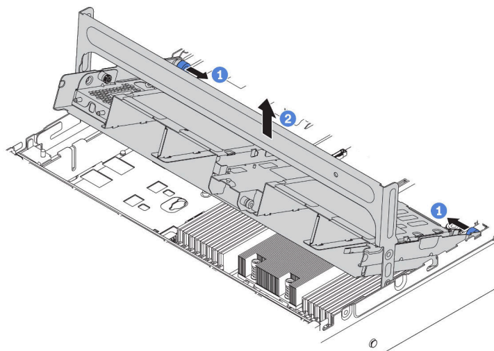
圖例 175. 卸下中間 2.5 吋框架
