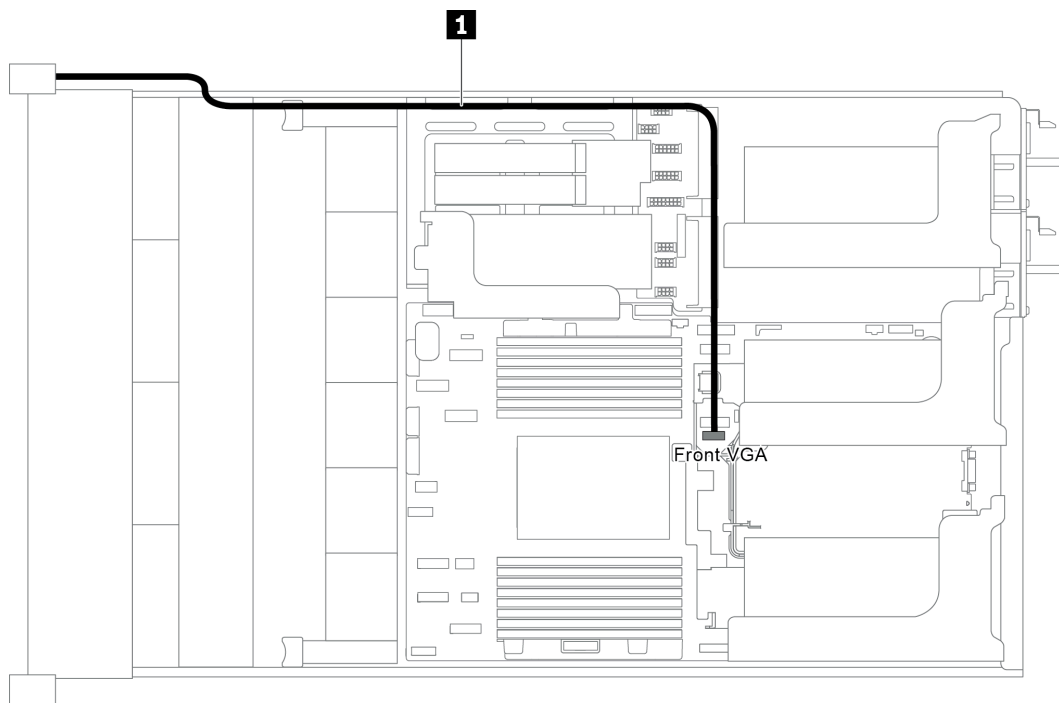
圖例 23. VGA 接頭纜線佈線
