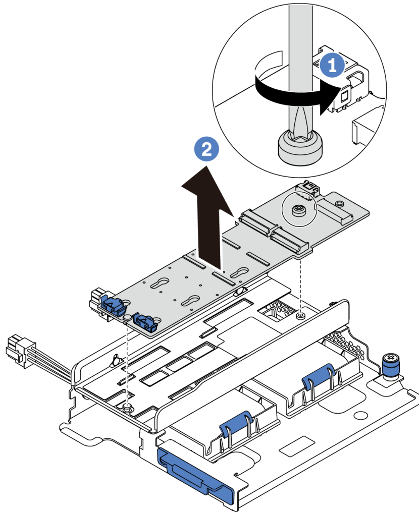
圖例 144. 卸下 M.2 配接卡
