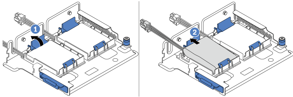
圖例 132. 卸下超級電容器模組
