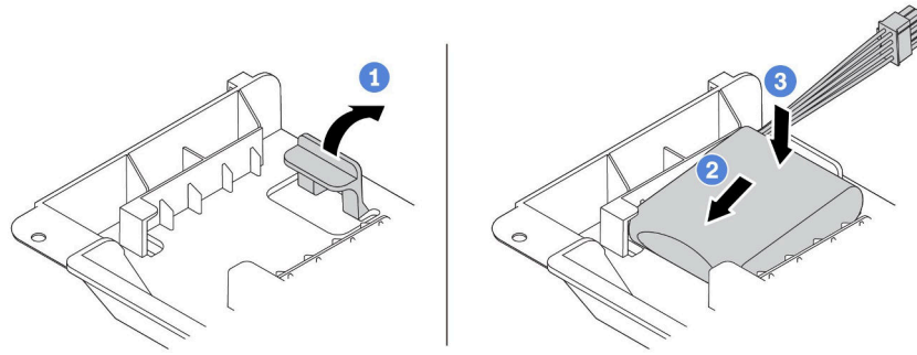
圖例 128. 空氣擋板上的超級電容器安裝
