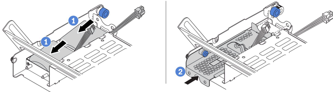
圖例 131. 中間 2.5 吋框架上的超級電容器安裝
