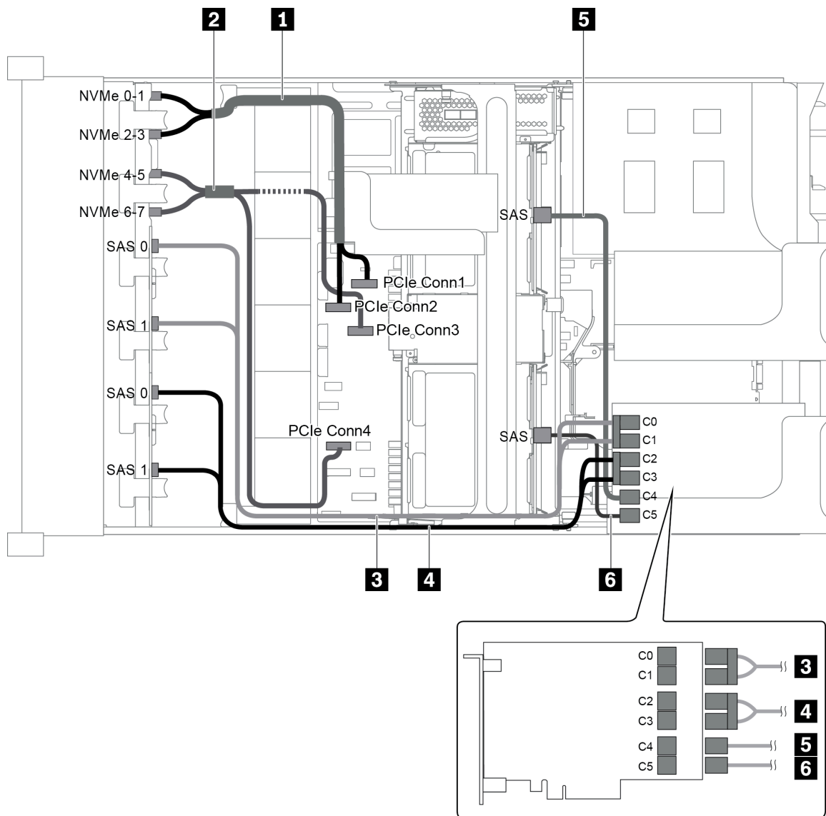
圖例 92. 配置為三個前方背板 (8 NVMe + 2 x 8 SAS/SATA)、一個中間框架和一張 24i RAID 配接卡的纜線佈線
