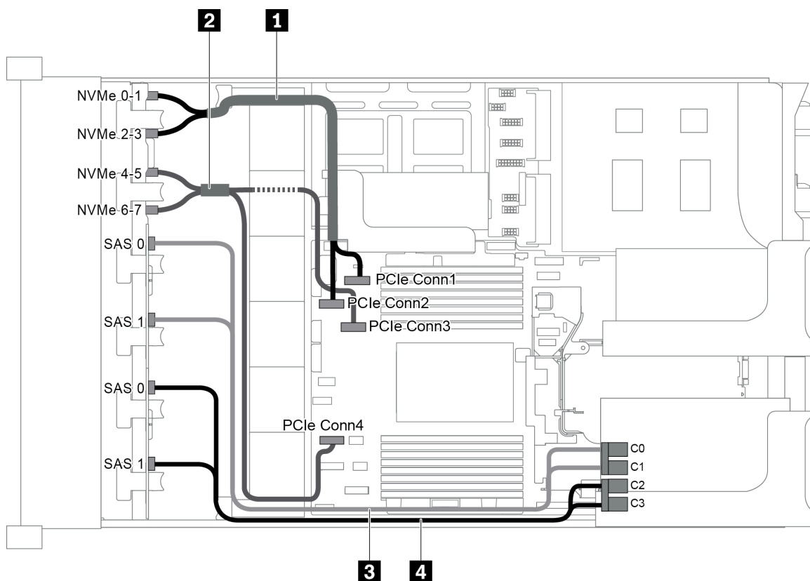
圖例 87. 配置為三個前方背板 (8 NVMe + 2 x 8 SAS/SATA) 和一張 16i RAID/HBA 配接卡的纜線佈線
