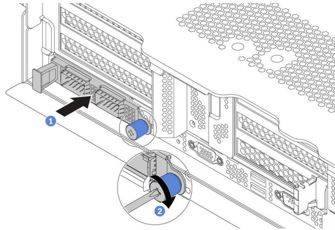
圖例 226. OCP 3.0 乙太網路配接卡安裝
