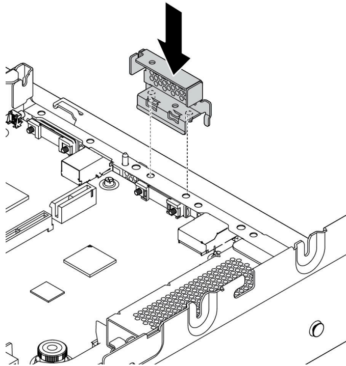
圖例 233. 安裝背面 3.5 吋框架的後壁托架
