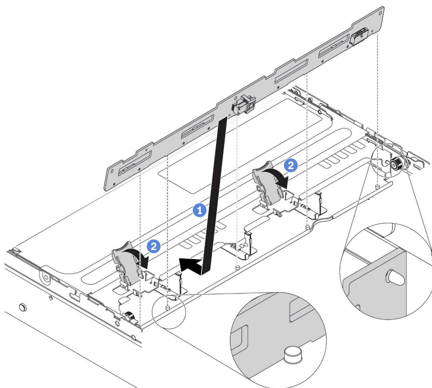
圖例 172. 安裝中間或後方 3.5 吋硬碟背板
