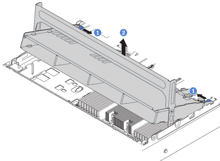
圖例 182. 卸下中間 3.5 吋框架
