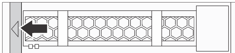
圖例 159. 打開 3.5 吋熱抽換硬碟的硬碟匣把手
