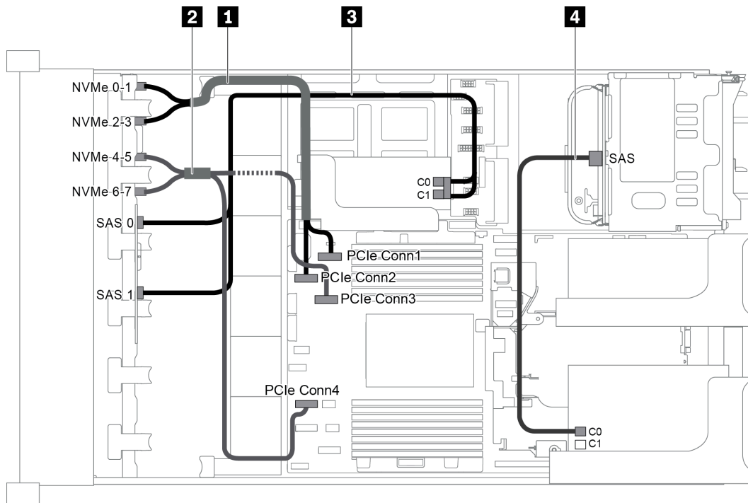
圖例 72. 配置為兩個前方背板 (8 NVMe + 8 SAS/SATA)、一個背面框架 (SAS/SATA) 和兩張 8i RAID/HBA 配接卡的纜線佈線
