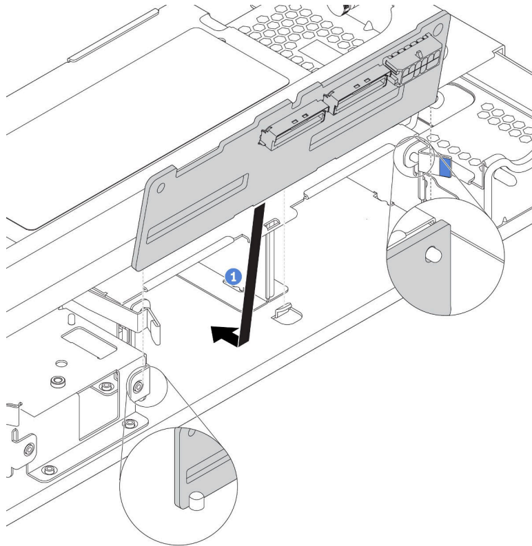
圖例 170. 安裝中間或後方 2.5 吋硬碟背板
