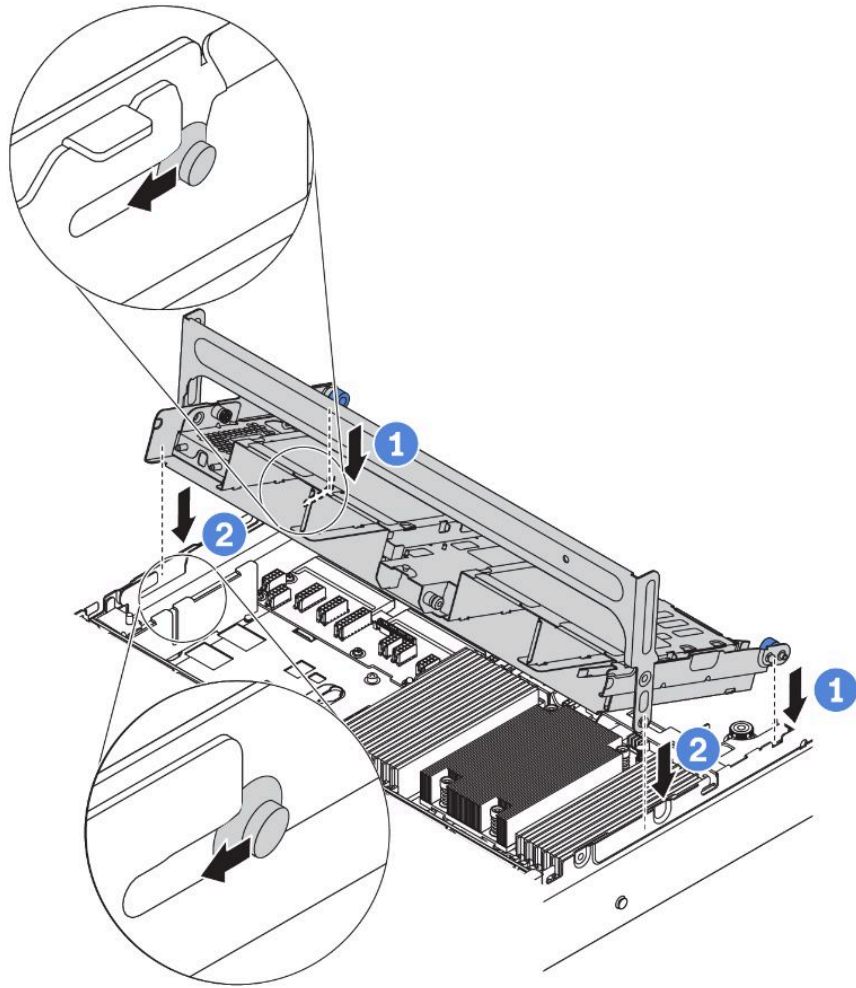
圖例 177. 安裝中間 2.5 吋框架
