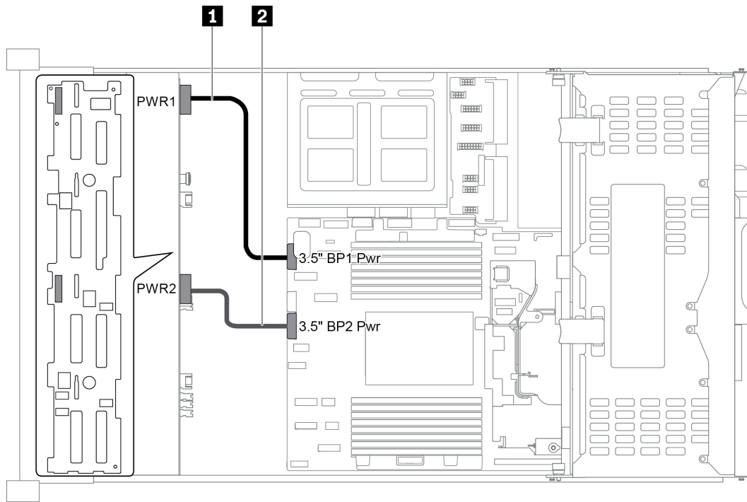
圖例 38. 前方 3.5 吋硬碟背板的電源佈線
