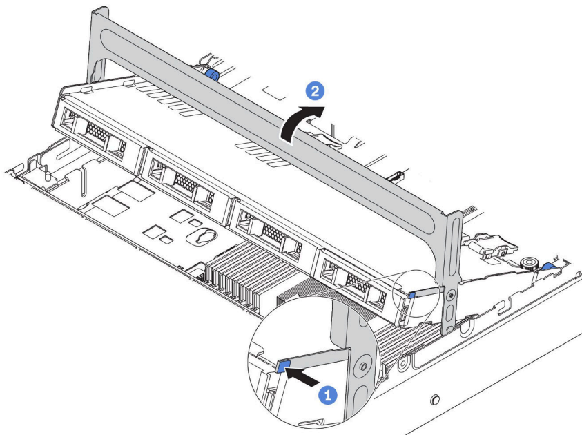
圖例 186. 關上框架把手
