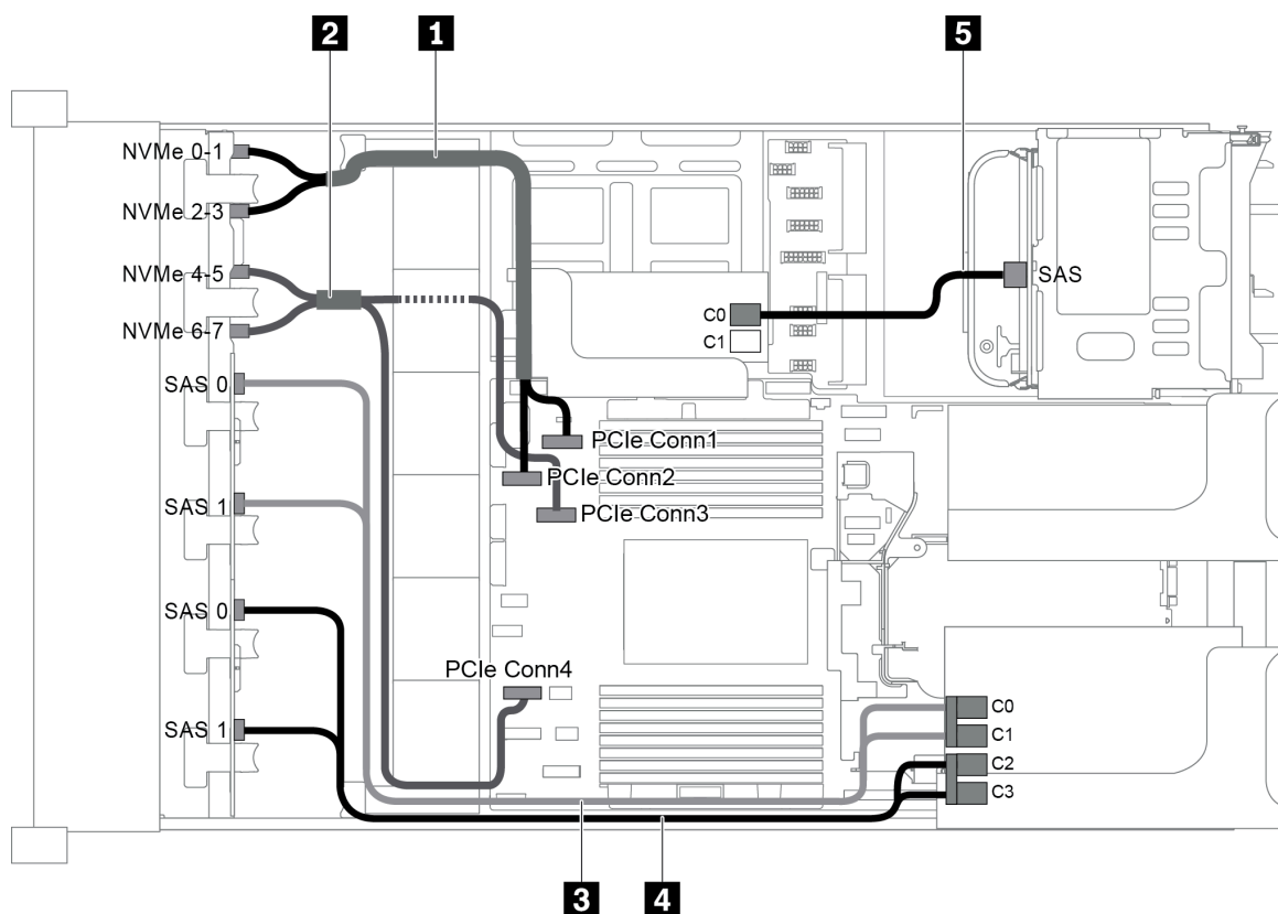
圖例 90. 配置為三個前方背板 (8 NVMe + 2 x 8 SAS/SATA)、一個背面框架和兩張 RAID/HBA 配接卡 (8i+16i) 的纜線佈線
