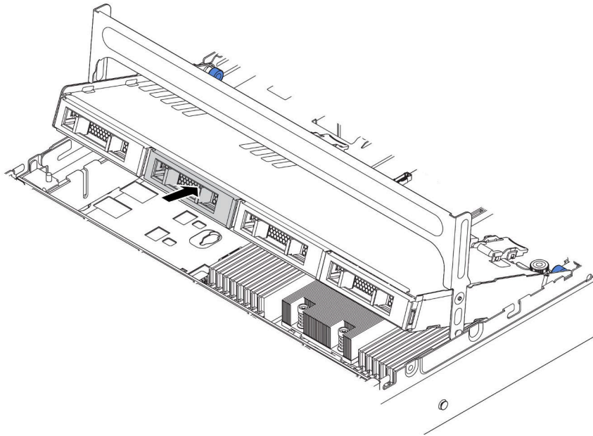
圖例 185. 將硬碟裝入框架
