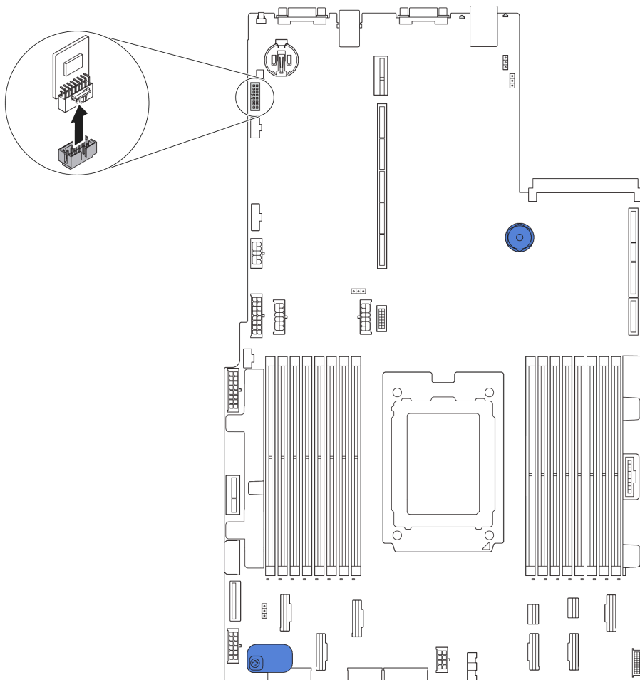
圖例 223. 卸下 TPM 配接卡
