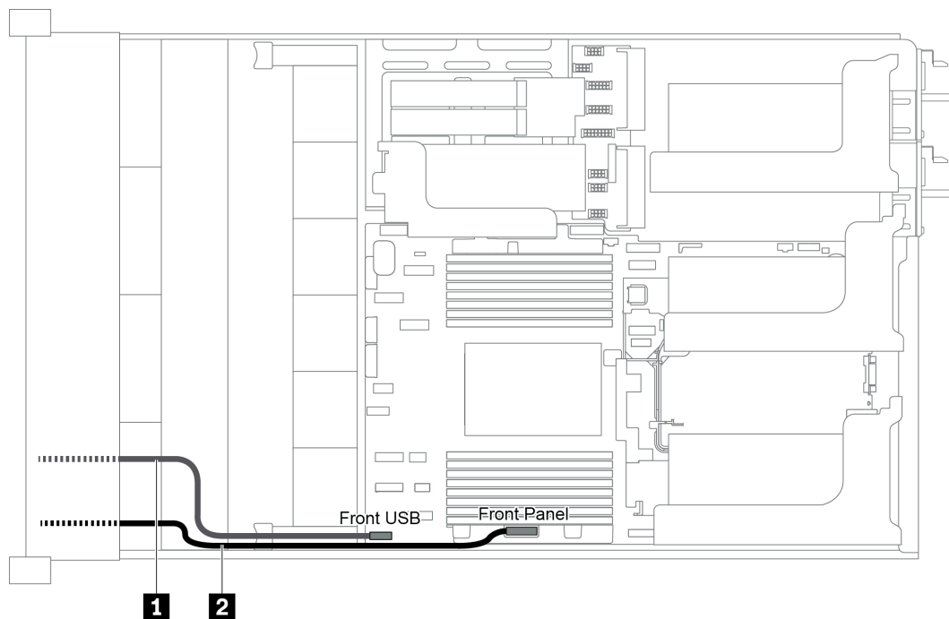
圖例 24. 機箱上正面 I/O 組件的纜線佈線
