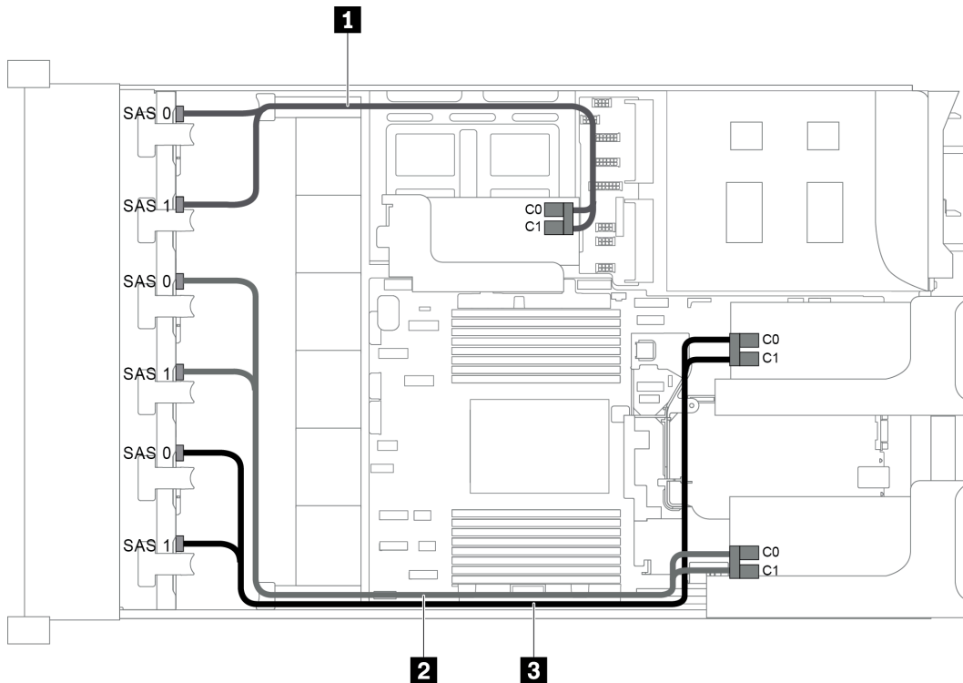
圖例 78. 配置為三個 8 x 2.5 吋 SAS/SATA 前方背板和三張 8i RAID/HBA 配接卡的纜線佈線
