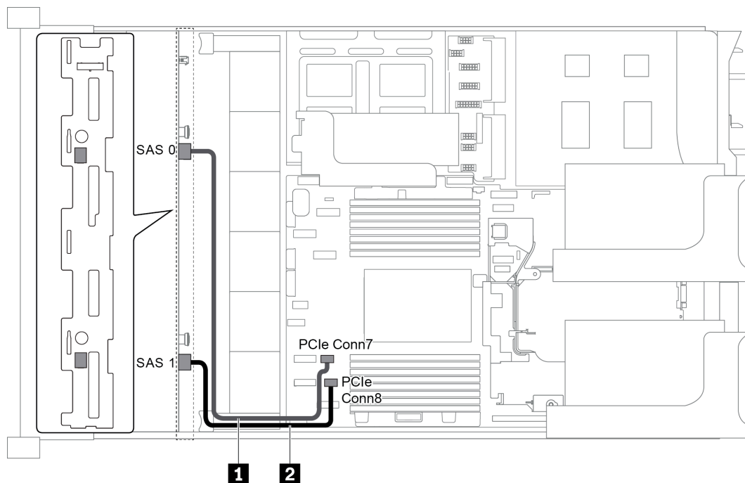
圖例 43. 配置為一個 8 x 3.5 吋 SAS/SATA 前方背板的纜線佈線
