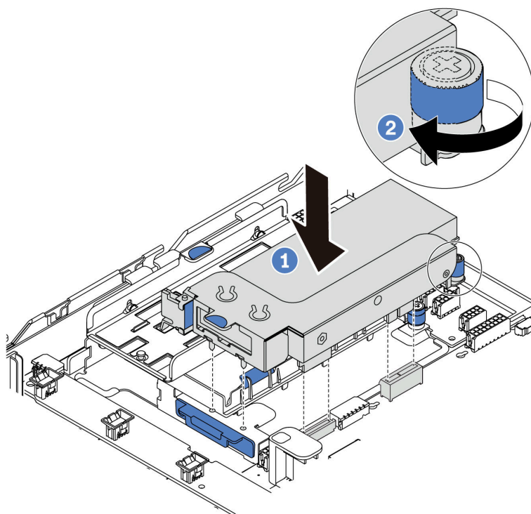
圖例 142. 內部擴充卡組件安裝
