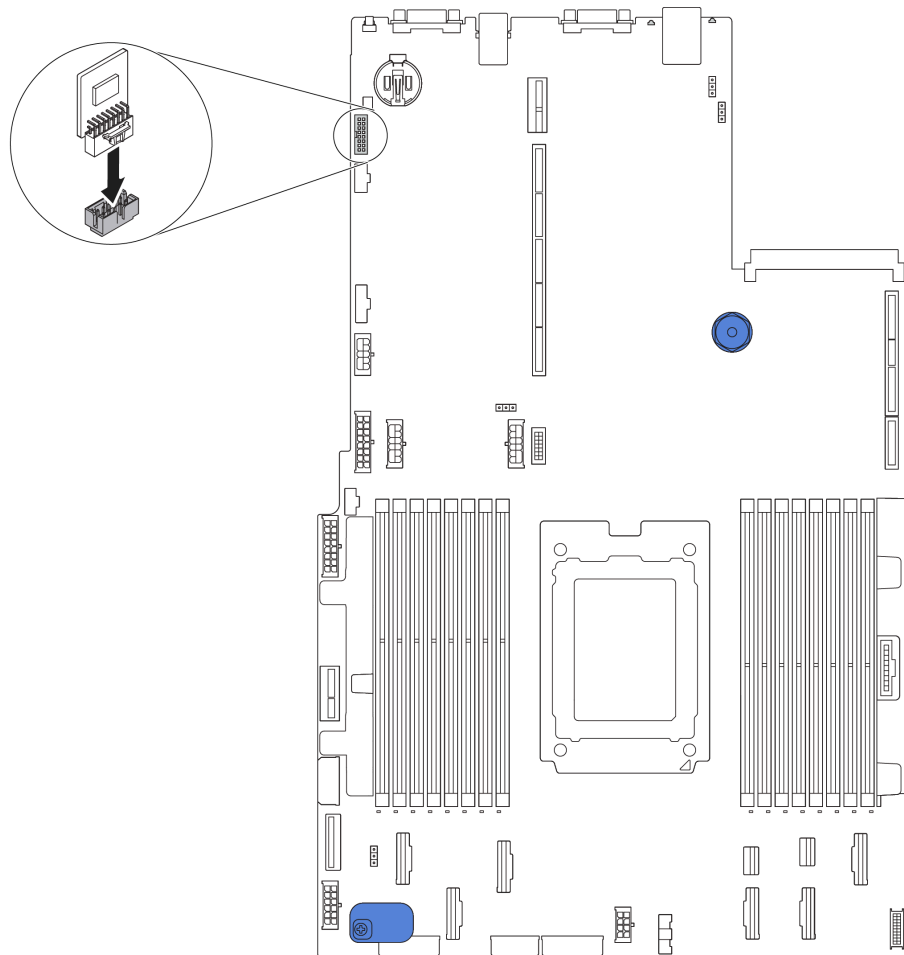
圖例 224. TPM 配接卡安裝
