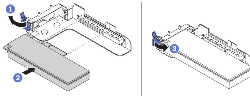
圖例 141. PCIe 配接卡安裝
