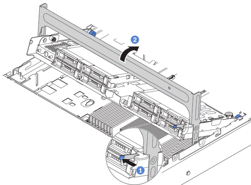
圖例 179. 關上框架把手
