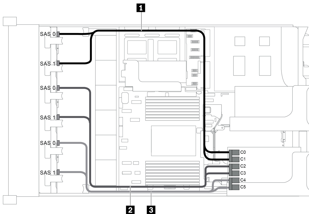
圖例 76. 配置為三個 8 x 2.5 吋 SAS/SATA 前方背板和一張 24i RAID 配接卡的纜線佈線
