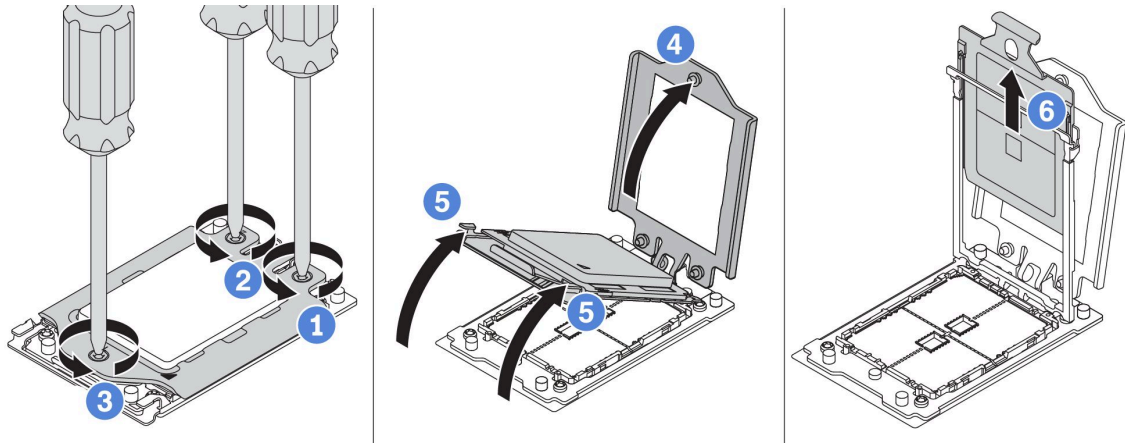
圖例 243. 卸下處理器
