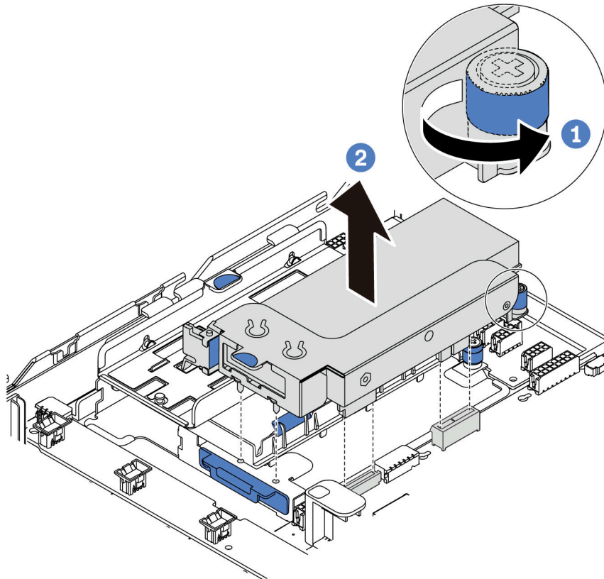
圖例 137. 卸下內部擴充卡組件
