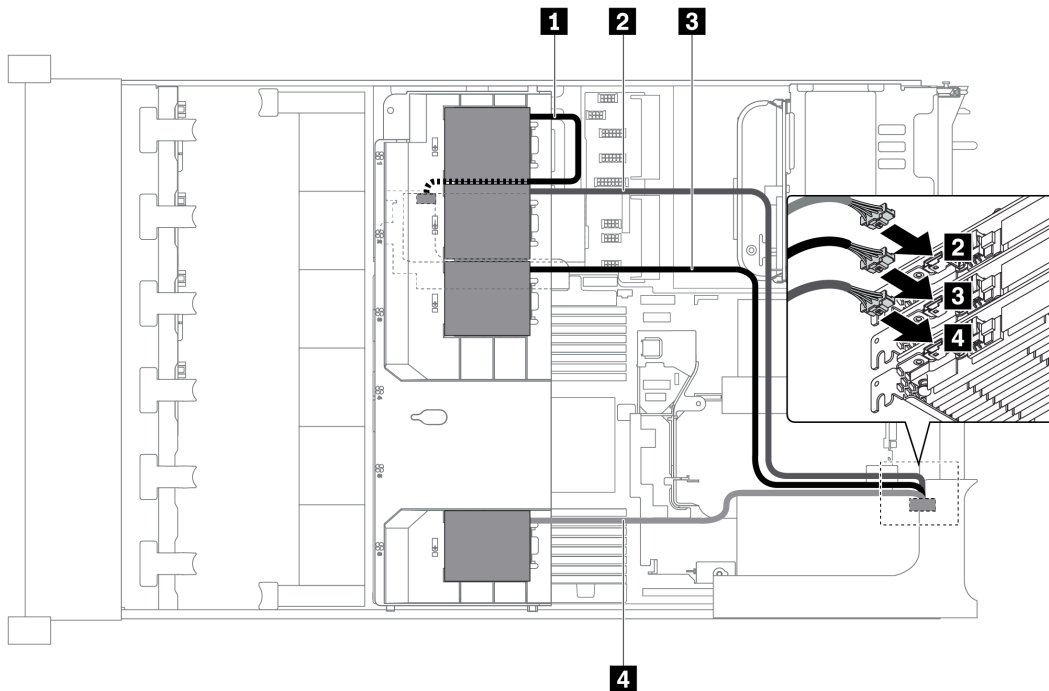
圖例 28. 標準空氣擋板上 RAID 超級電容器模組的纜線佈線
