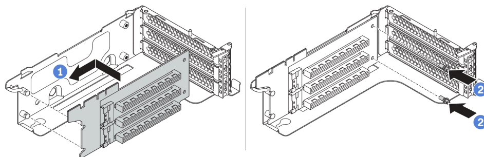
圖例 201. 擴充卡安裝
