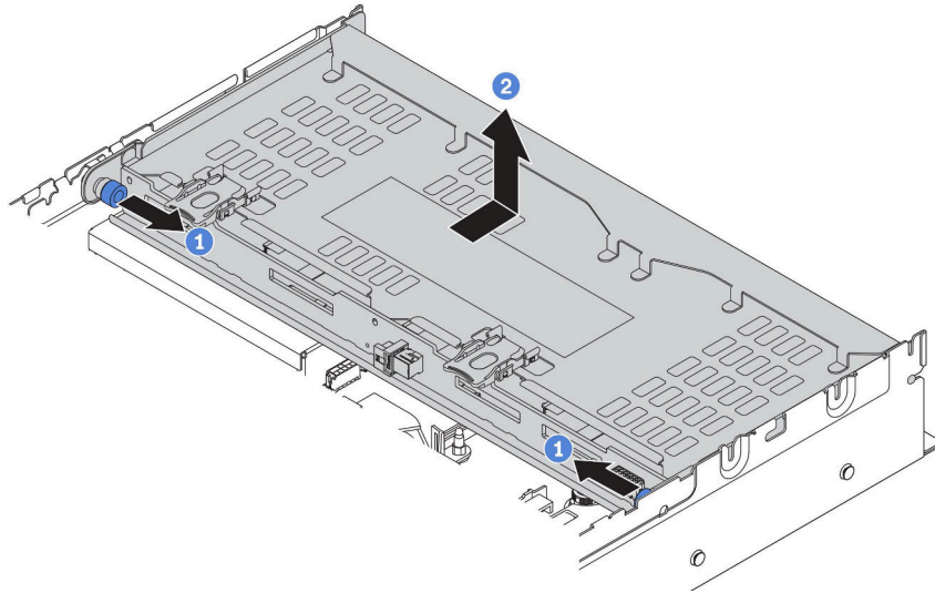
圖例 232. 卸下背面 3.5 吋框架
