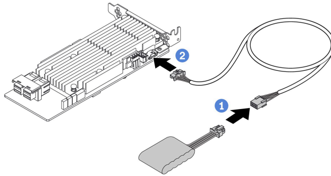
圖例 27. 將 RAID 超級電容器模組連接至 RAID 配接卡
