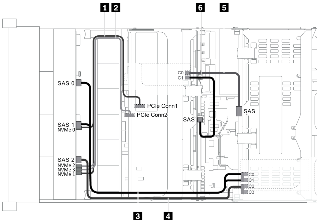
圖例 58. 配置為一個 12 x 3.5 吋 AnyBay 前方背板、一個後方框架、一個中間框架和兩張 RAID/HBA 配接卡 (8i+16i) 的纜線佈線
