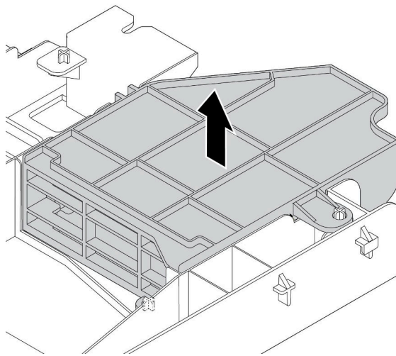
圖例 220. 卸下單倍寬 GPU 配接卡適用的 GPU 空氣擋板附加元件
