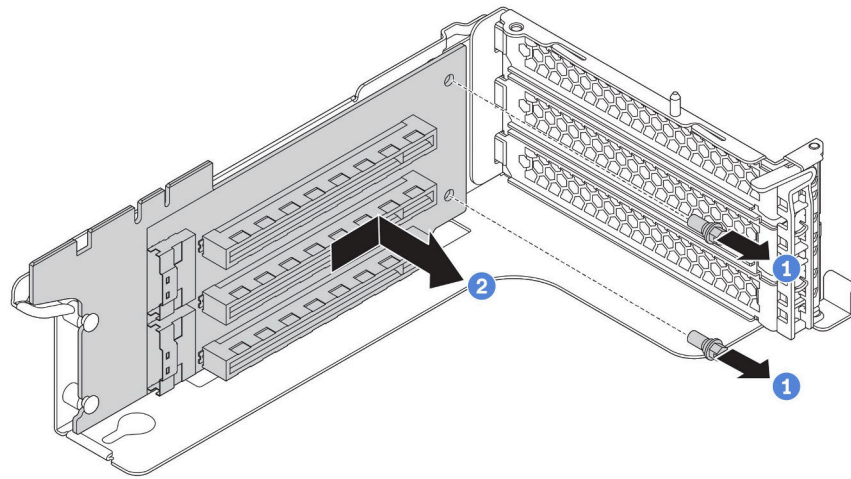
圖例 194. 卸下擴充卡
