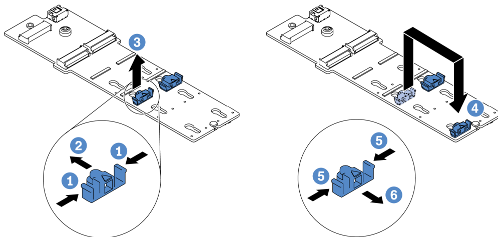
圖例 146. 調整 M.2 固定器
