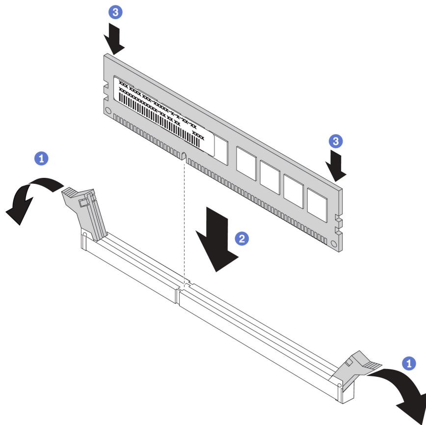
圖例 188. 安裝記憶體模組
