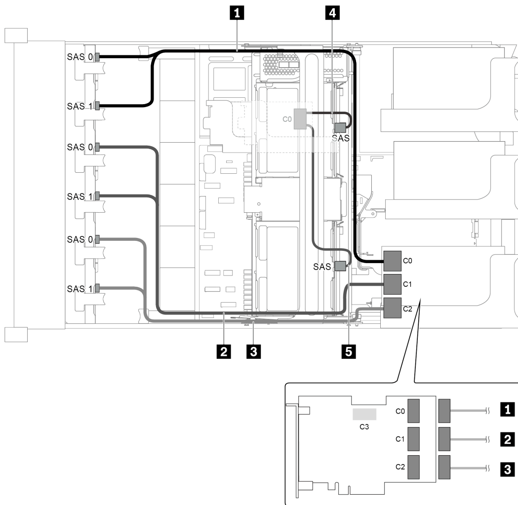
圖例 85. 配置為三個 8 x 2.5 吋 SAS/SATA 前方背板、一個中間框架和兩張 RAID/HBA 配接卡 (8i+32i) 的纜線佈線
