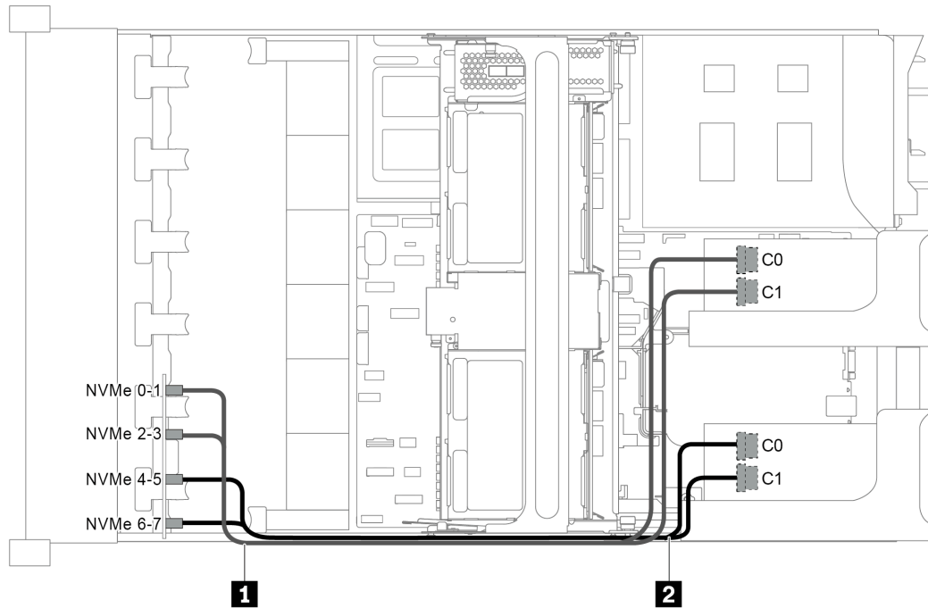
圖例 105. 配置為前方背板上的兩個 NVMe 重定時器配接卡的纜線佈線
