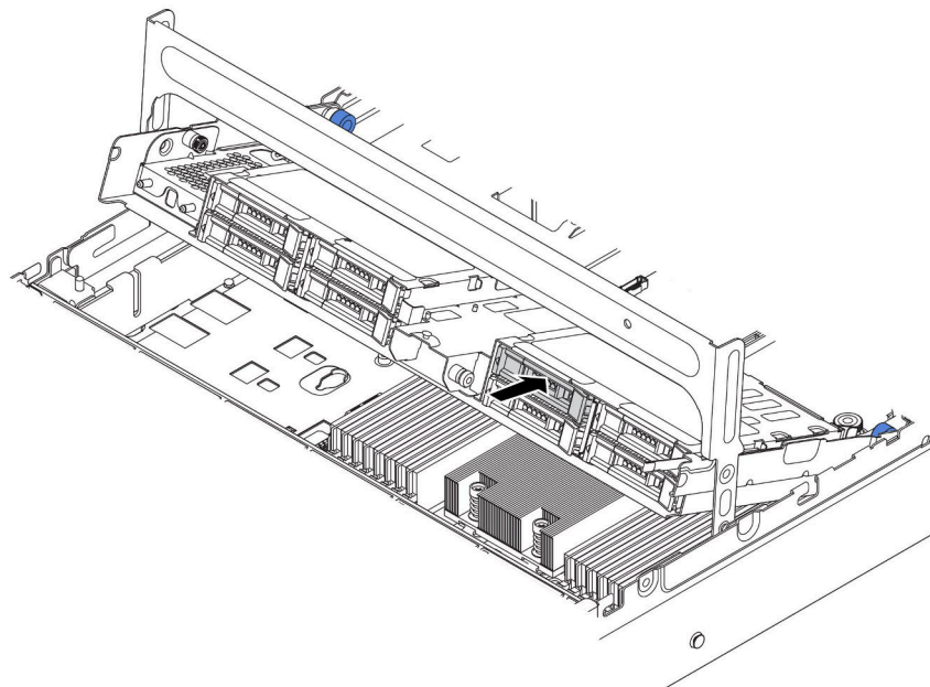
圖例 178. 將硬碟裝入框架
