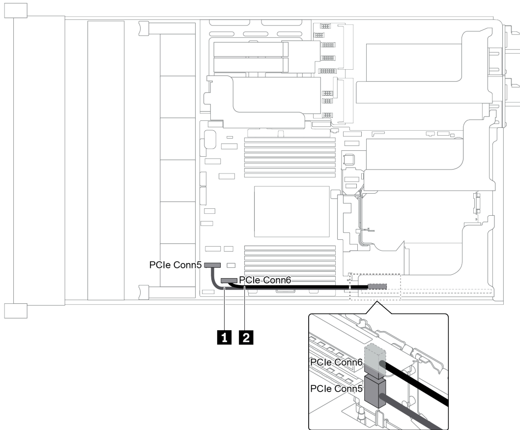
圖例 33. 擴充卡 1 的纜線佈線
