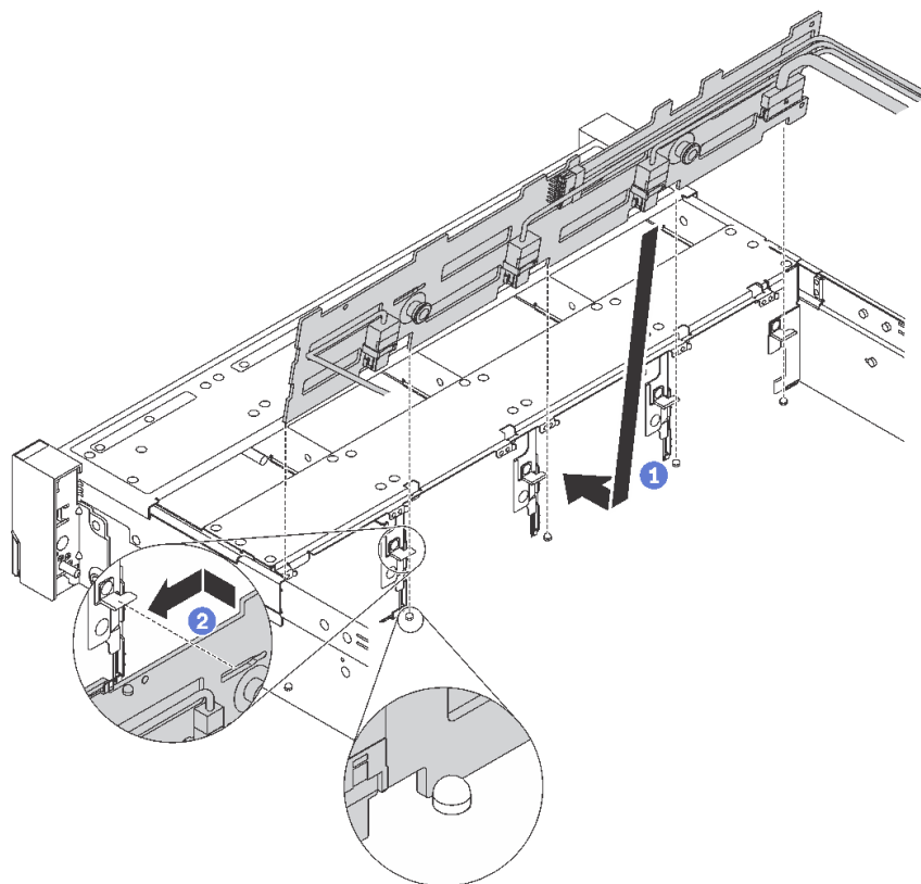
圖例 168. 3.5 吋硬碟背板安裝
