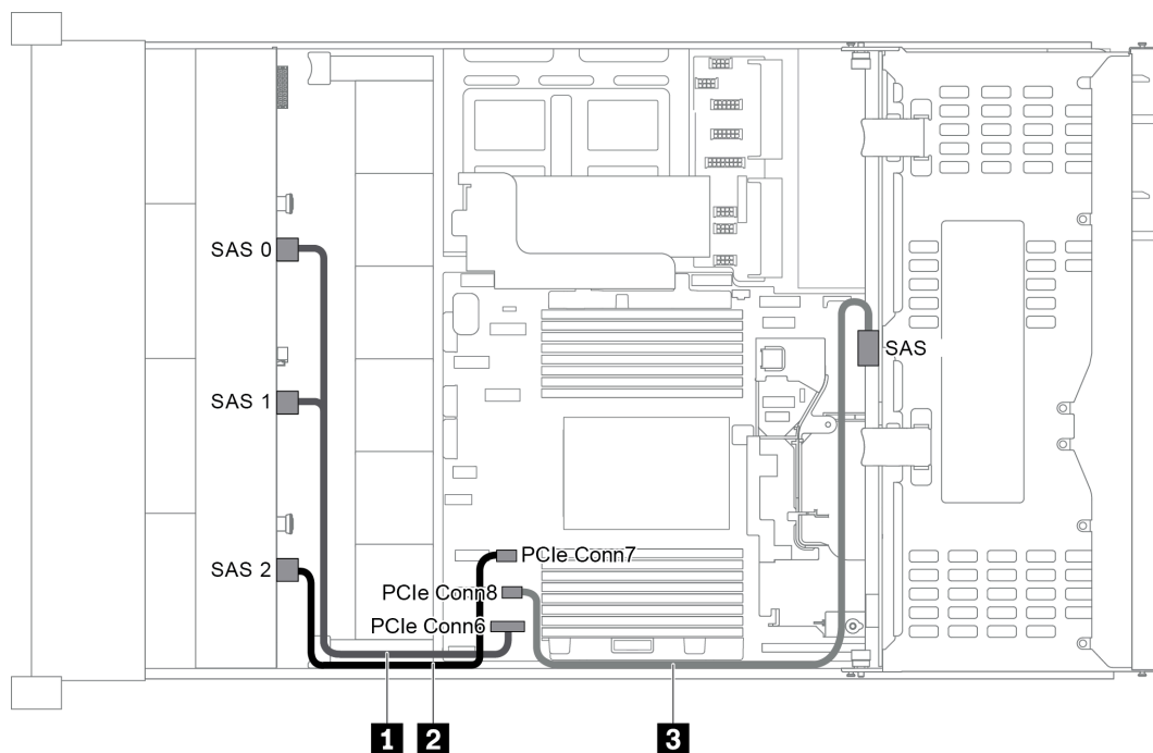
圖例 47. 配置為一個 12 x 3.5 吋 SAS/SATA 前方背板和一個背面框架 (SAS/SATA) 的纜線佈線
