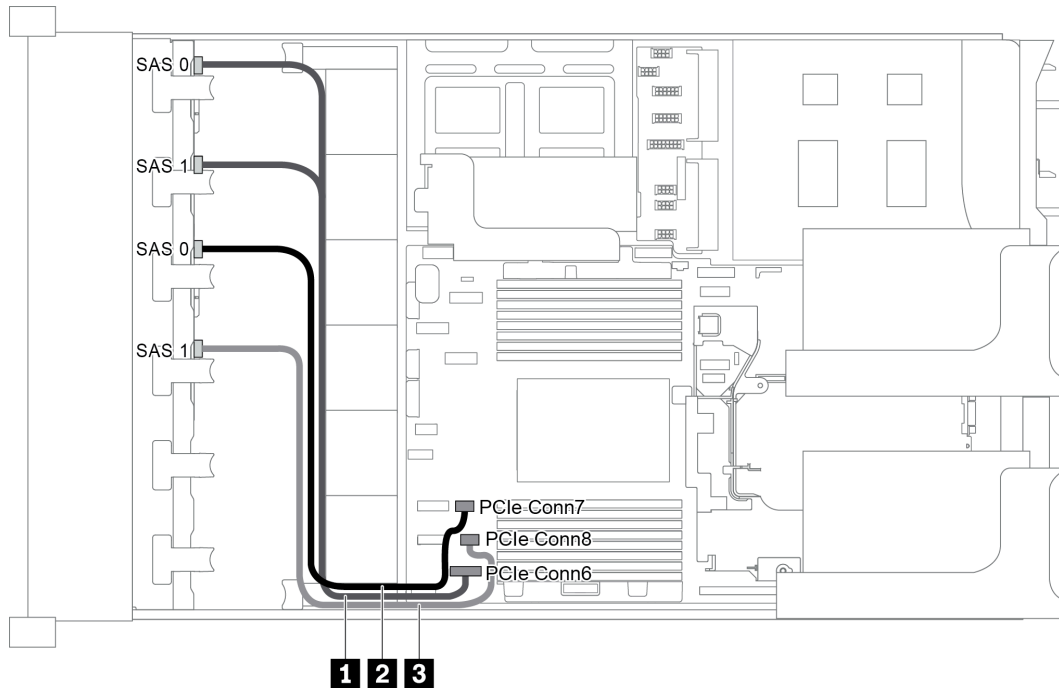
圖例 62. 配置為兩個 8 x 2.5 吋 SAS/SATA 前方背板的纜線佈線
