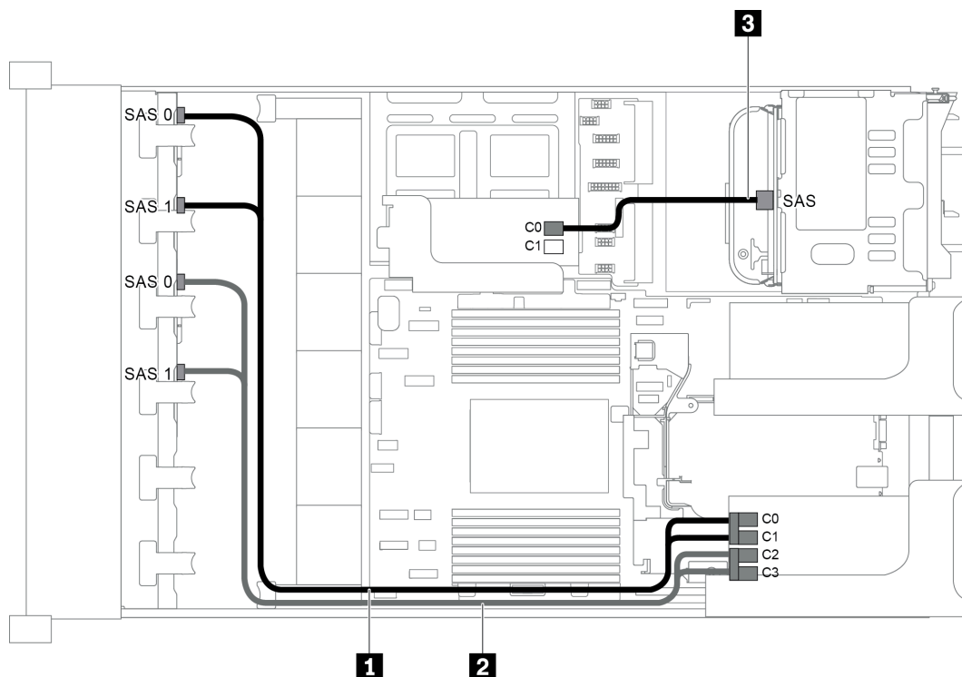
圖例 66. 配置為兩個 8 x 2.5 吋 SAS/SATA 前方背板、一個背面框架和兩張 RAID/HBA 配接卡 (8i+16i) 的纜線佈線
