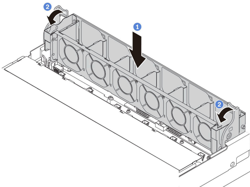
圖例 155. 系統風扇機盒安裝
