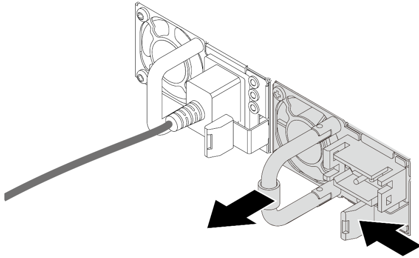
圖例 237. 卸下熱抽換電源供應器
