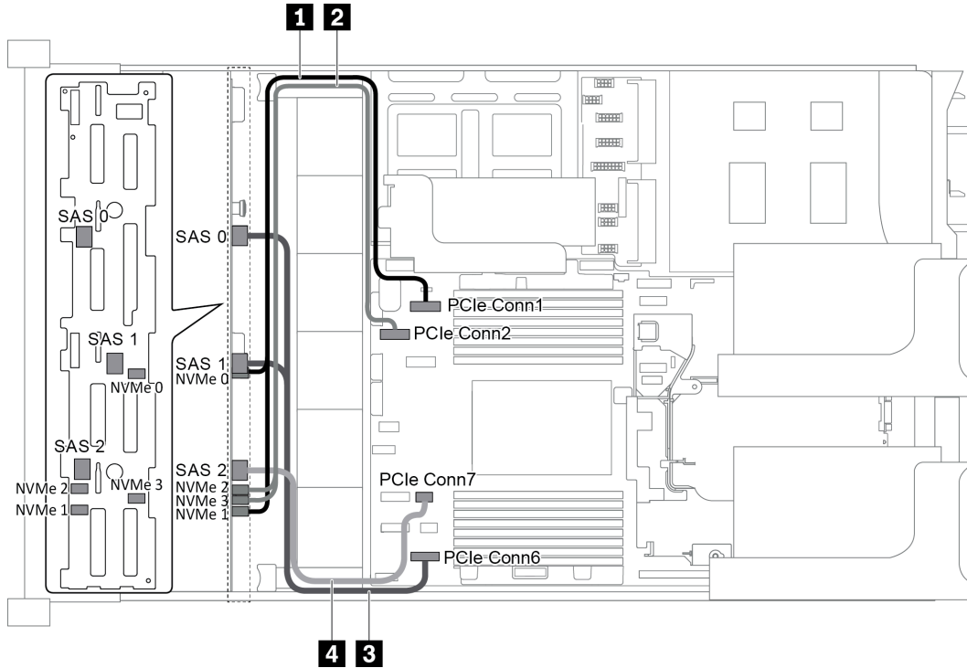
圖例 53. 配置為一個 12 x 3.5 吋 AnyBay 前方背板的纜線佈線
