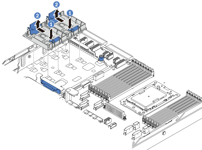
圖例 133. 卸下超級電容器固定器
