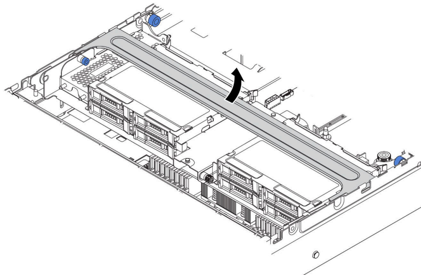
圖例 173. 打開框架把手
