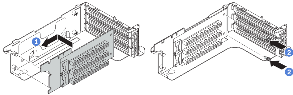
圖例 205. 擴充卡安裝
