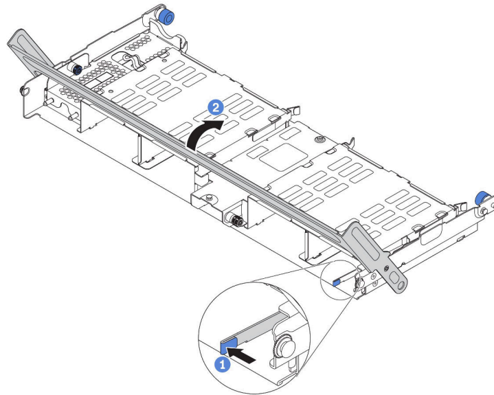
圖例 176. 合上中間 2.5 吋框架的把手
