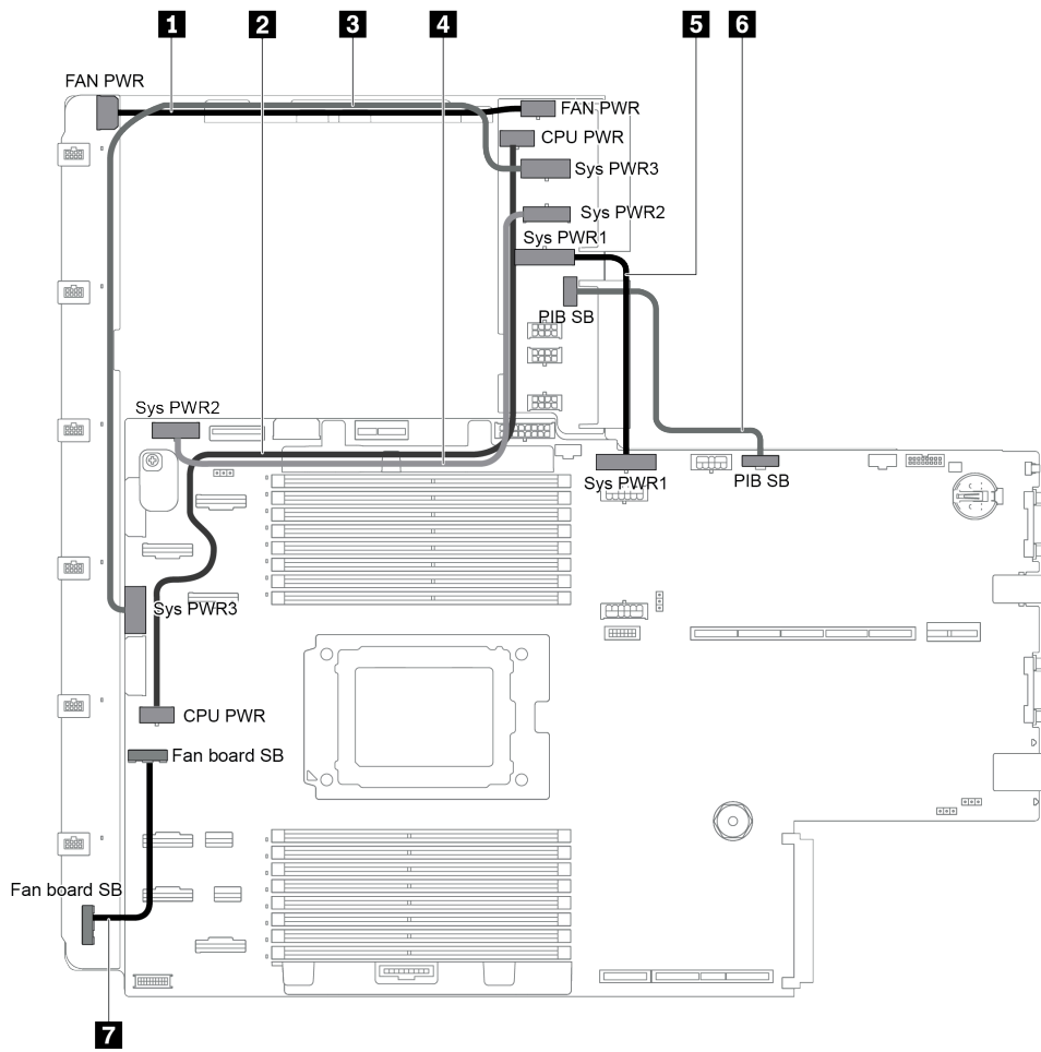
圖例 108. 主機板、PIB 板和風扇板之間的連線
