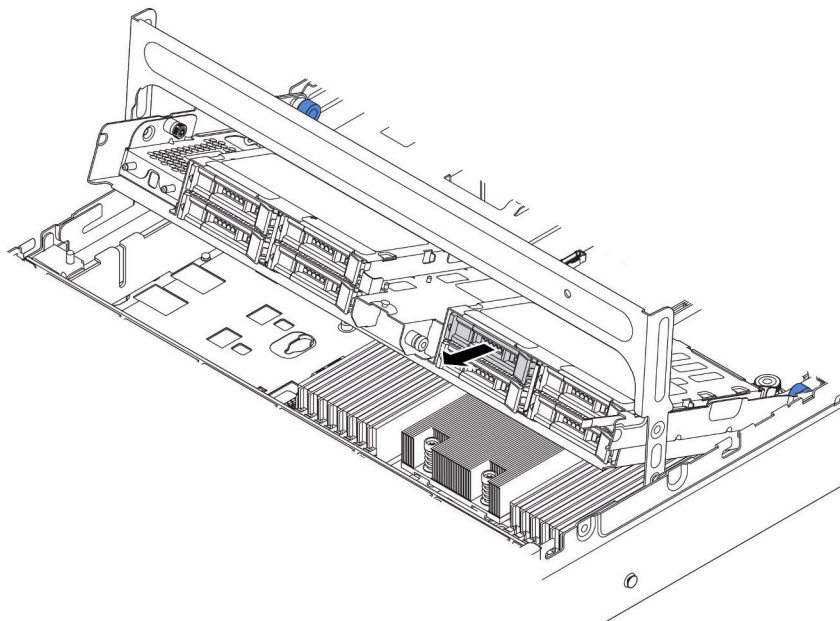
圖例 174. 從中間 2.5 吋框架卸下硬碟
