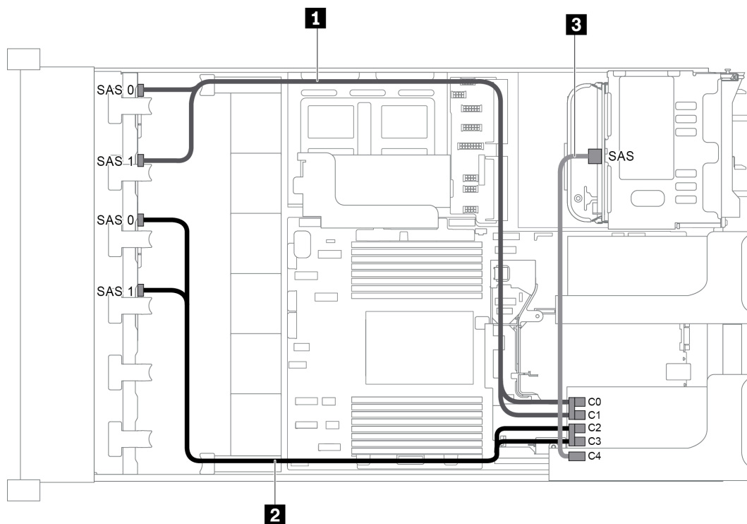
圖例 65. 配置為兩個 8 x 2.5 吋 SAS/SATA 前方背板、一個背面框架和一張 24i RAID 配接卡的纜線佈線
