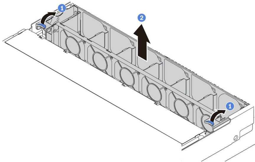
圖例 154. 卸下系統風扇機盒
