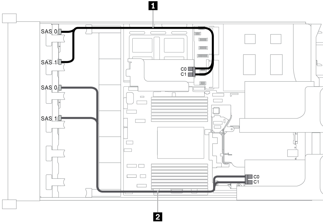
圖例 64. 配置為兩個 8 x 2.5 吋 SAS/SATA 前方背板和兩張 8i RAID/HBA 配接卡的纜線佈線
