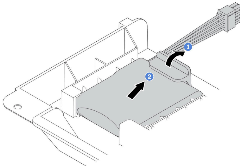
圖例 127. 卸下超級電容器模組
