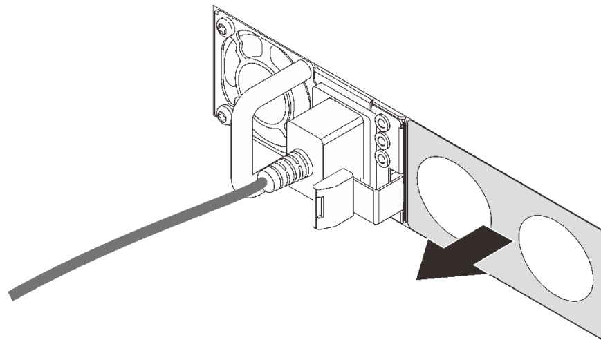
圖例 240. 卸下熱抽換電源供應器填充板
