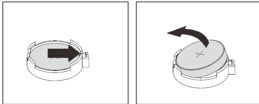
圖例 189. 卸下 CMOS 電池
