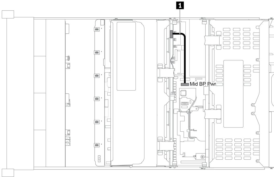
圖例 40. 中間 3.5 吋硬碟背板的電源佈線
