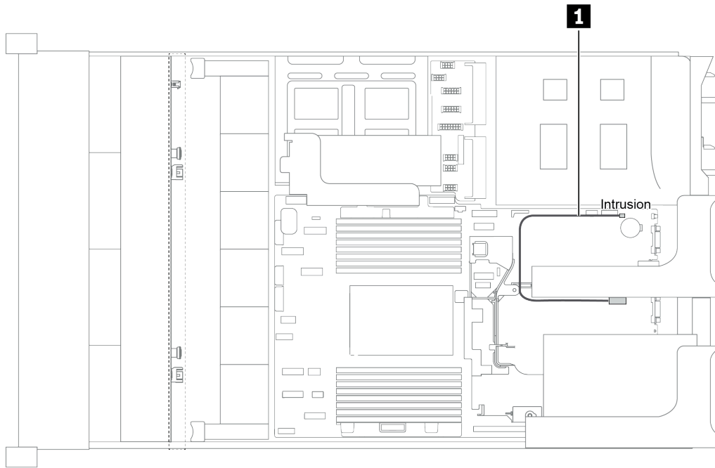
圖例 32. 入侵開關纜線佈線
