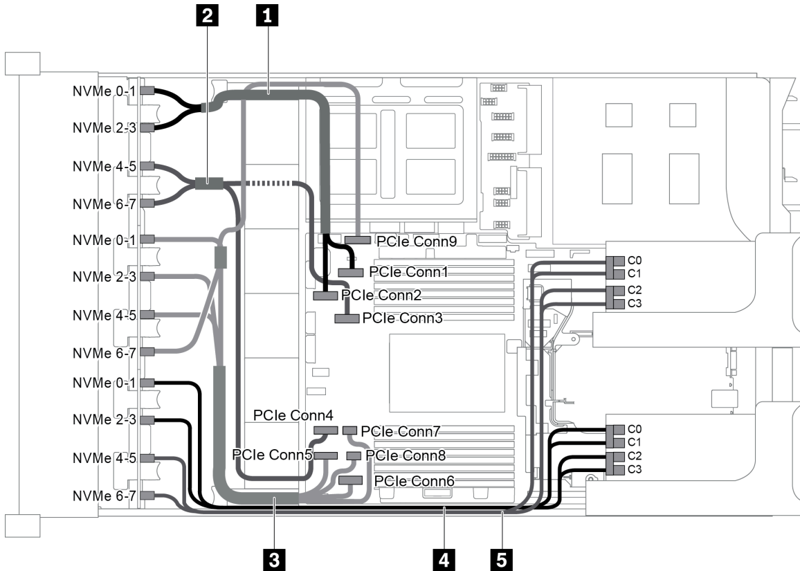
圖例 97. 配置為三個 8 x 2.5 吋 NVMe 前方背板和兩張 810-4P 或 1610-4P NVMe 交換器卡的纜線佈線
