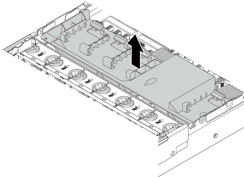
圖例 112. 卸下標準空氣擋板
