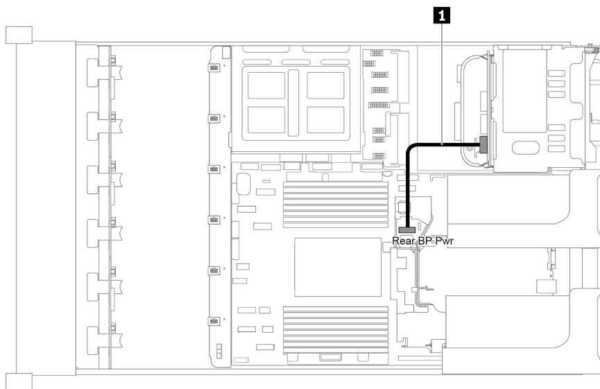
圖例 40. 後方 2.5 吋硬碟背板的電源佈線
