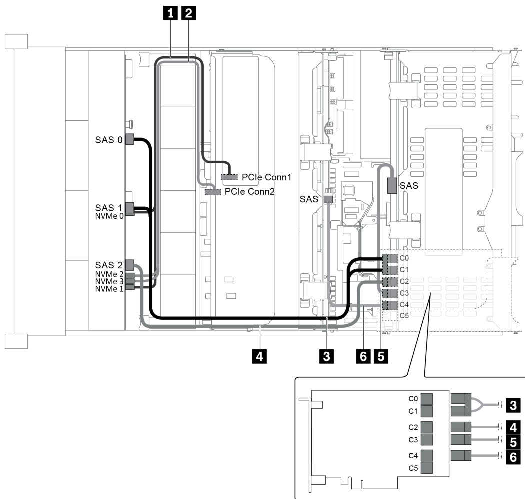
圖例 56. 配置為一個 12 x 3.5 吋 AnyBay 前方背板、一個後方框架、一個中間框架和一張 24i RAID 配接卡的纜線佈線
