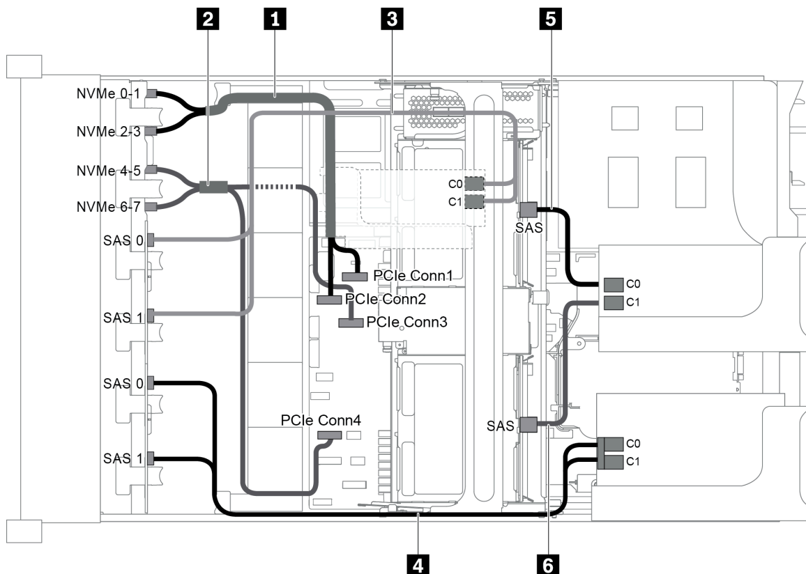
圖例 93. 配置為三個前方背板 (8 NVMe + 2 x 8 SAS/SATA)、一個中間框架和三張 8i RAID/HBA 配接卡的纜線佈線
