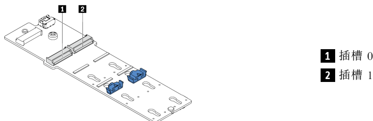
圖例 124. M.2 硬碟插槽
