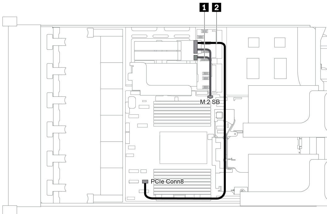
圖例 25. M.2 硬碟的纜線佈線
