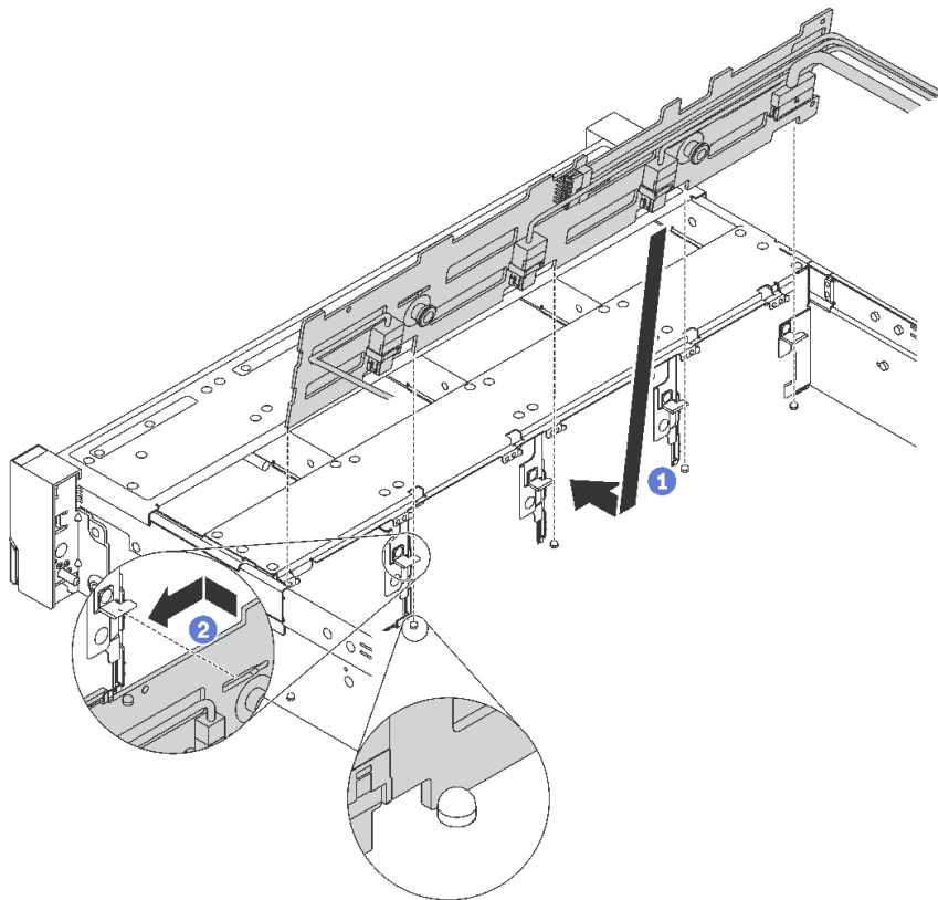
圖例 130. 3.5 吋硬碟背板安裝
