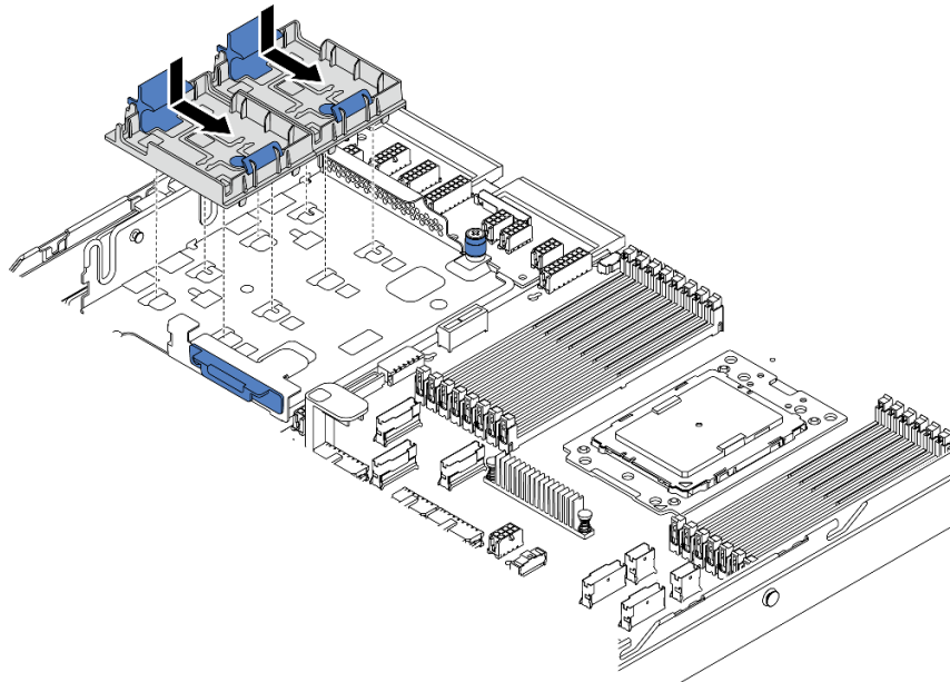
圖例 118. 超級電容器固定器安裝
