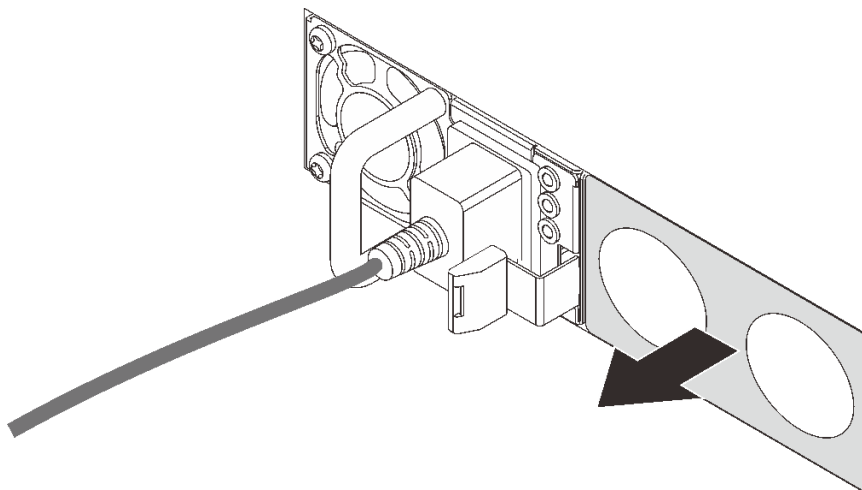
圖例 156. 卸下熱抽換電源供應器填充板
