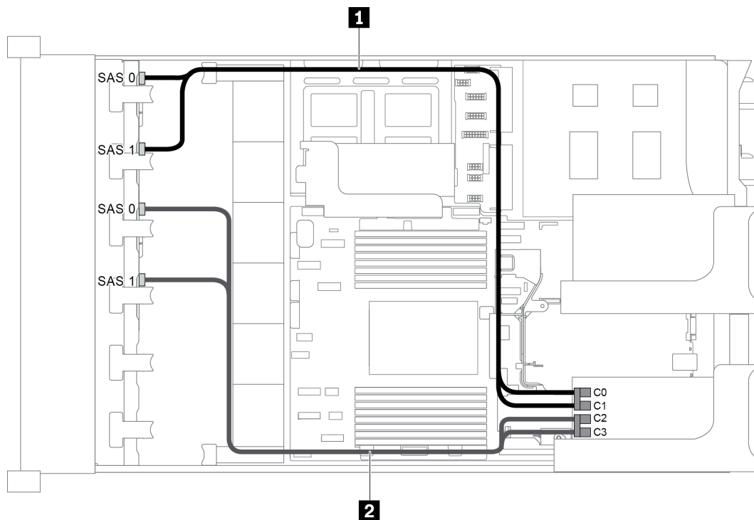
圖例 62. 配置為兩個 8 x 2.5 吋 SAS/SATA 前方背板和一張 16i RAID/HBA 配接卡的纜線佈線
