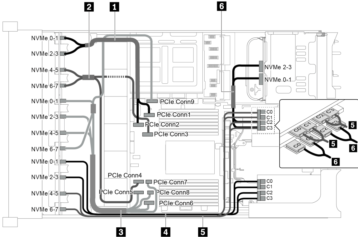
圖例 99. 配置為三個 8 x 2.5 吋 NVMe 前方背板、一個背面框架 (NVMe) 和三張 810-4P 或 1610-4P NVMe 交換器卡的纜線佈線
