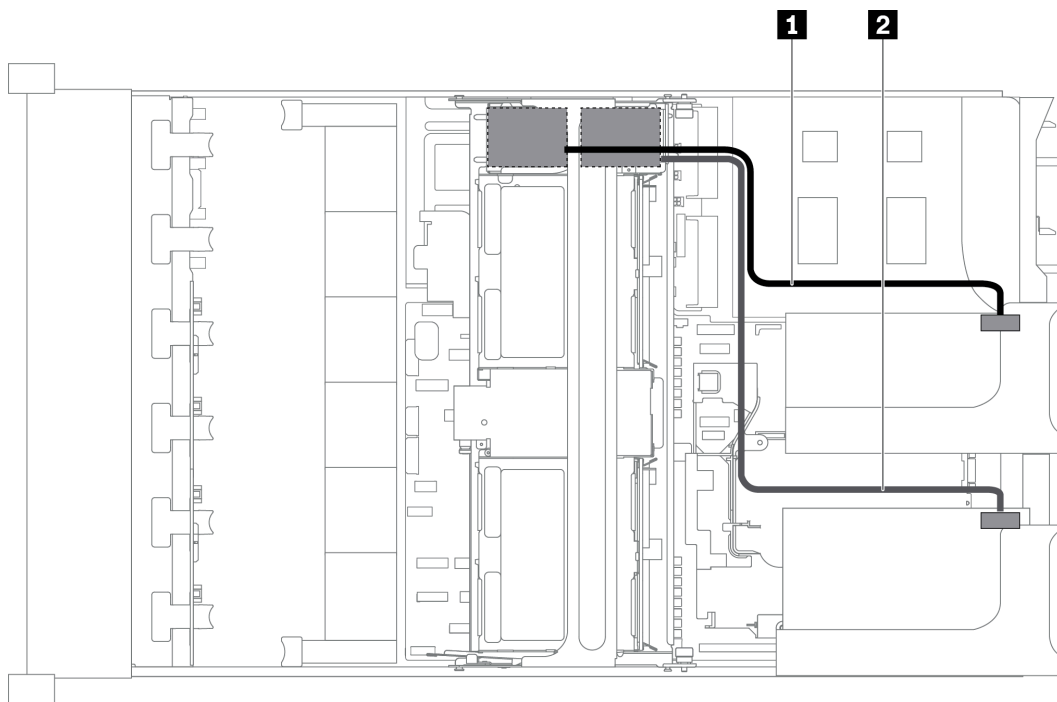
圖例 28. 中間框架上 RAID 超級電容器模組的纜線佈線
