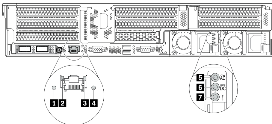
圖例 18. 伺服器的背面圖 LED
