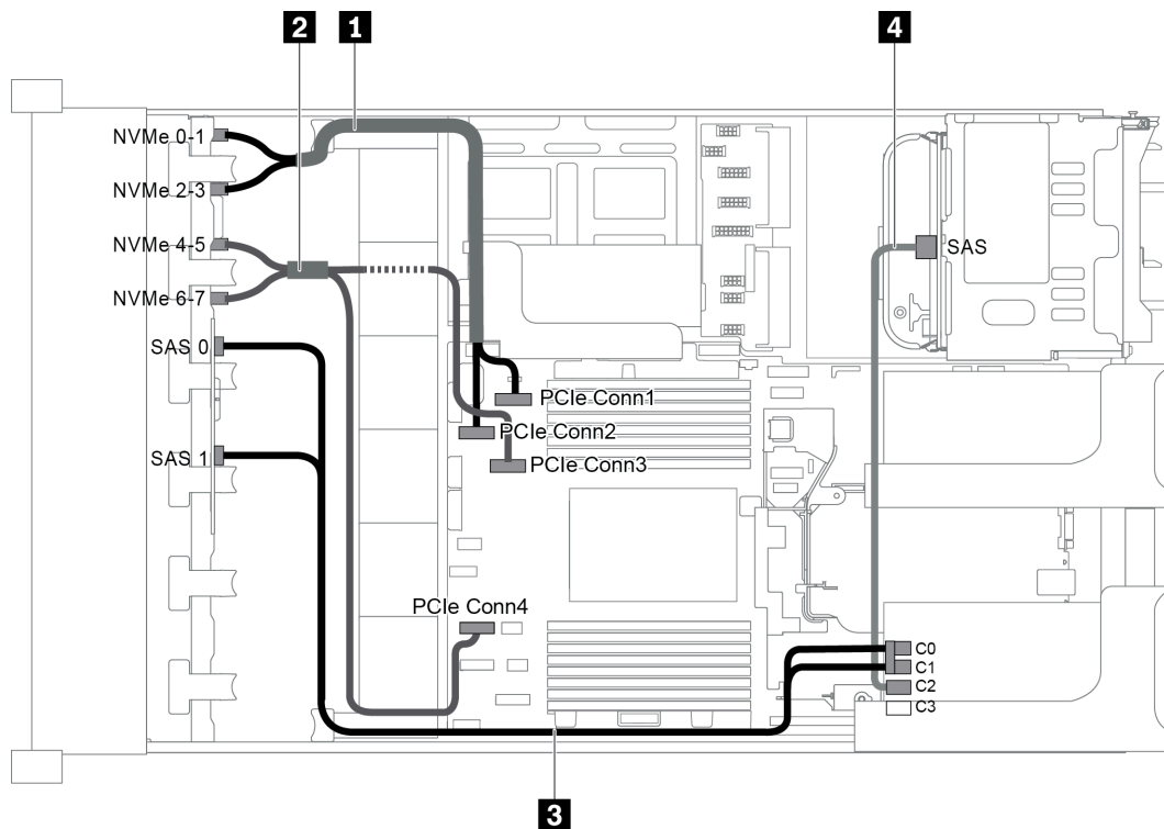
圖例 70. 配置為兩個前方背板 (8 NVMe + 8 SAS/SATA)、一個背面框架和一張 16i RAID/HBA 配接卡的纜線佈線
