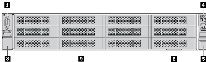
圖例 10. 未配備背板之伺服器型號
