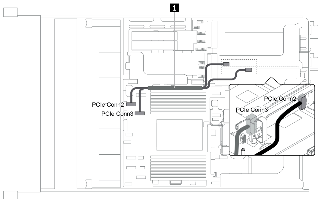
圖例 33. 擴充卡 3 (x8/x8 PCIe) 的纜線佈線
