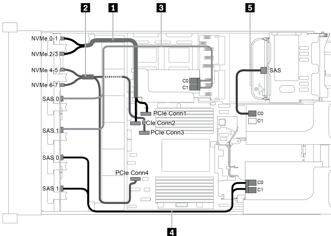
圖例 90. 配置為三個前方背板 (8 NVMe + 2 x 8 SAS/SATA)、一個後方框架和三張 8i RAID/HBA 配接卡的纜線佈線
