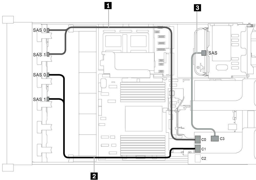
圖例 67. 配置為兩個 8 x 2.5 吋 SAS/SATA 前方背板、一個後方框架和一張 32i RAID 配接卡的纜線佈線
