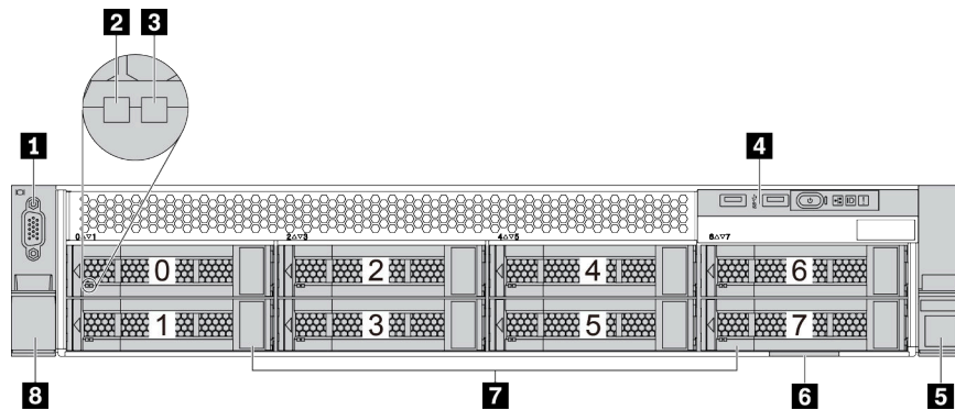
圖例 8. 配備八個 3.5 吋機槽的伺服器型號
