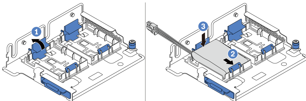
圖例 119. 超級電容器模組安裝
