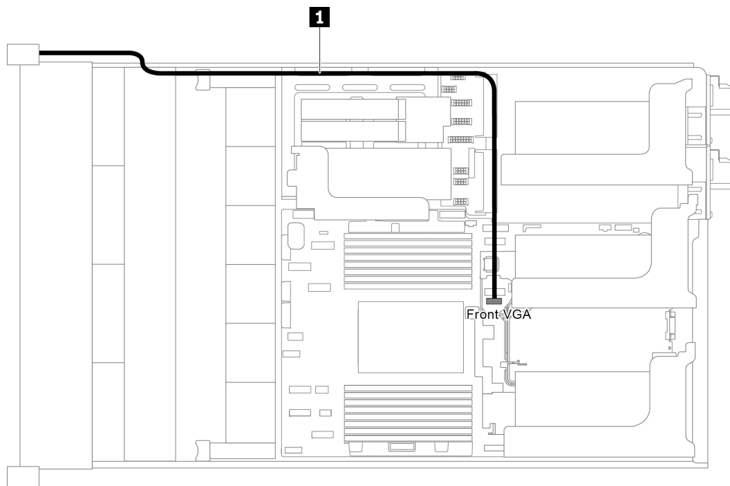
圖例 22. VGA 接頭纜線佈線
