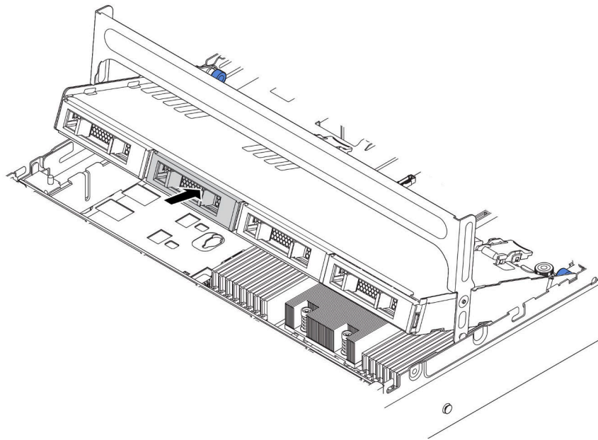
圖例 139. 將硬碟裝入框架
