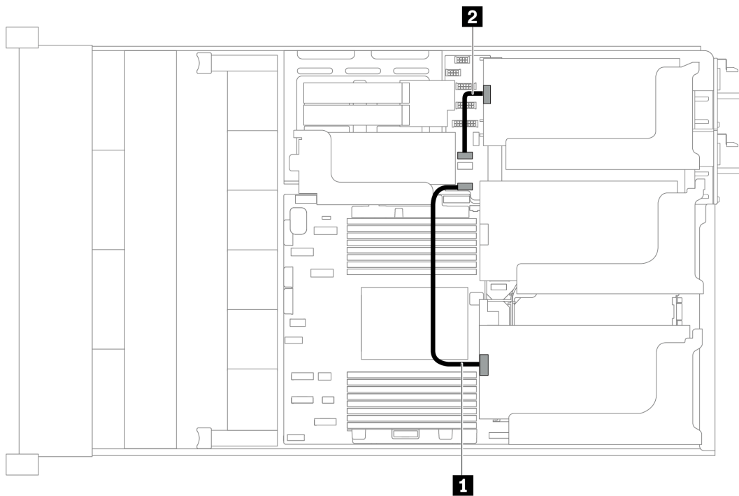
圖例 30. GPU 配接卡的纜線佈線
