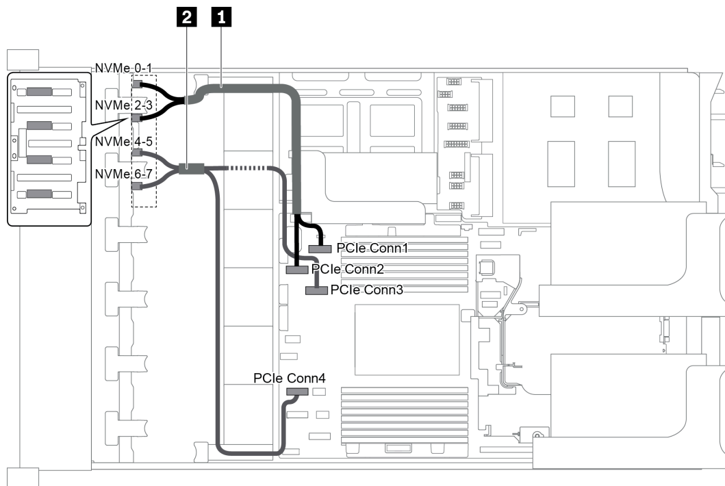
圖例 60. 配置為一個 8 x 2.5 吋 NVMe 前方背板的纜線佈線
