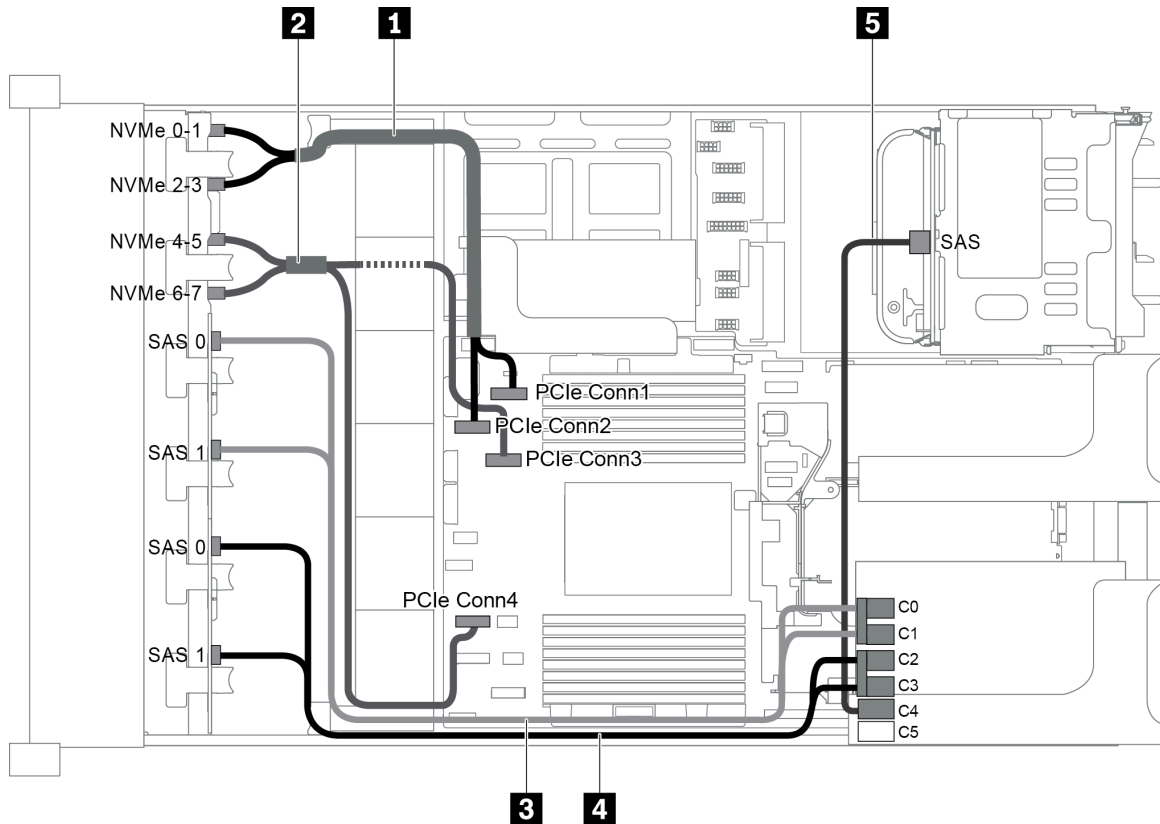
圖例 88. 配置為三個前方背板 (8 NVMe + 2 x 8 SAS/SATA)、一個背面框架和一張 24i RAID 配接卡的纜線佈線
