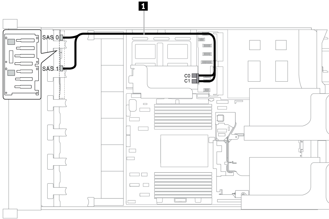
圖例 59. 配置為一個 8 x 2.5 吋 SAS/SATA 前方背板和一張 8i RAID/HBA 配接卡的纜線佈線
