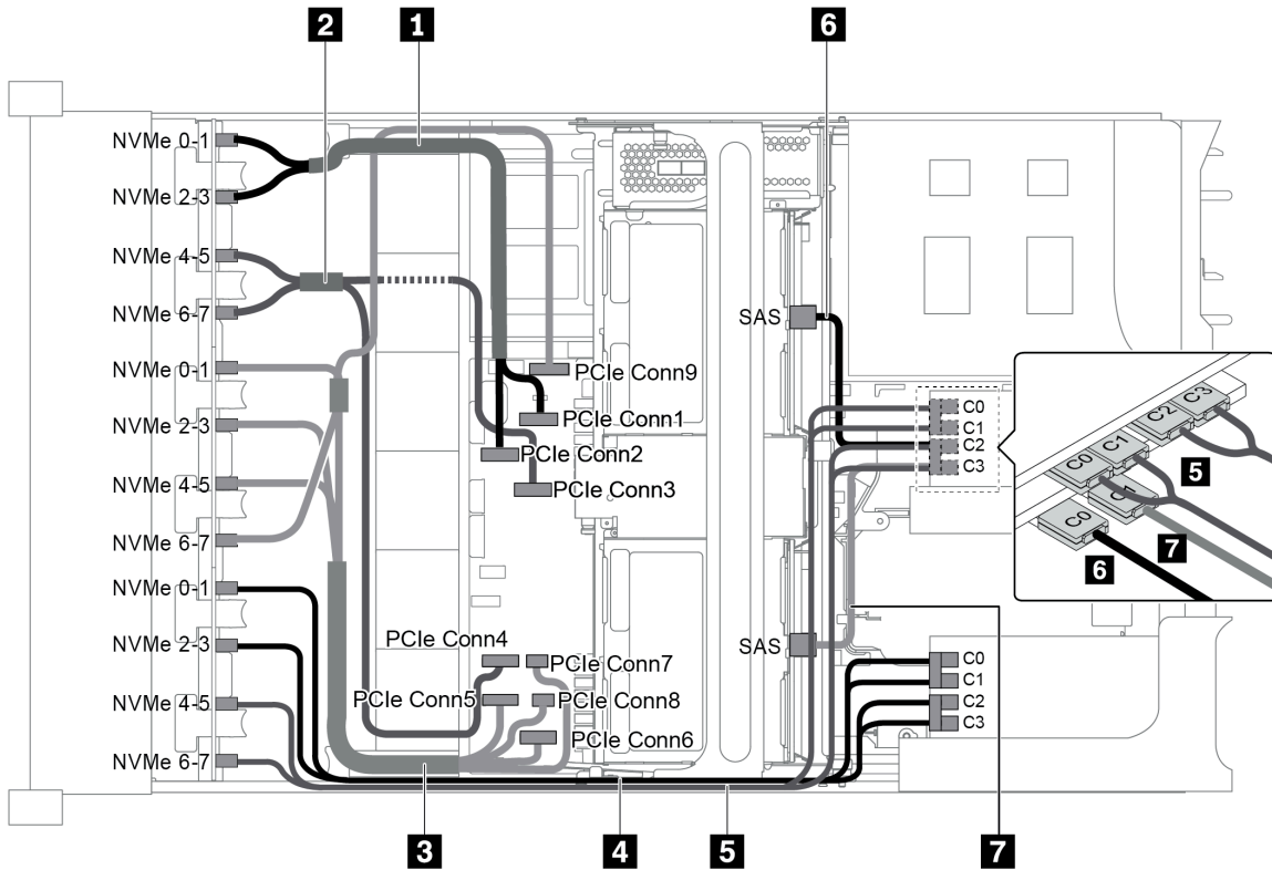
圖例 100. 配置為三個 8 x 2.5 吋 NVMe 前方背板、一個中間框架 (SAS/SATA)、兩張 810-4P 或 1610-4P NVMe 交換器卡和一張 8i RAID/HBA 配接卡的纜線佈線
