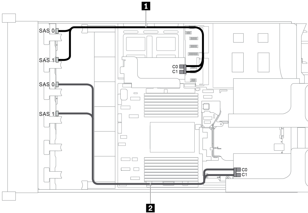
圖例 63. 配置為兩個 8 x 2.5 吋 SAS/SATA 前方背板和兩張 8i RAID/HBA 配接卡的纜線佈線
