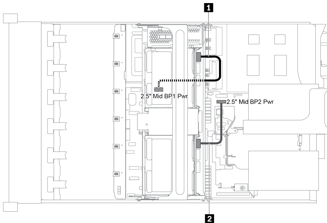
圖例 38. 中間 2.5 吋硬碟背板的電源佈線
