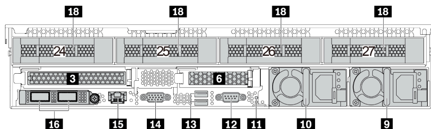
圖例 15. 配備 3.5 吋背面機槽和兩個 PCIe 插槽之伺服器型號的背面圖
