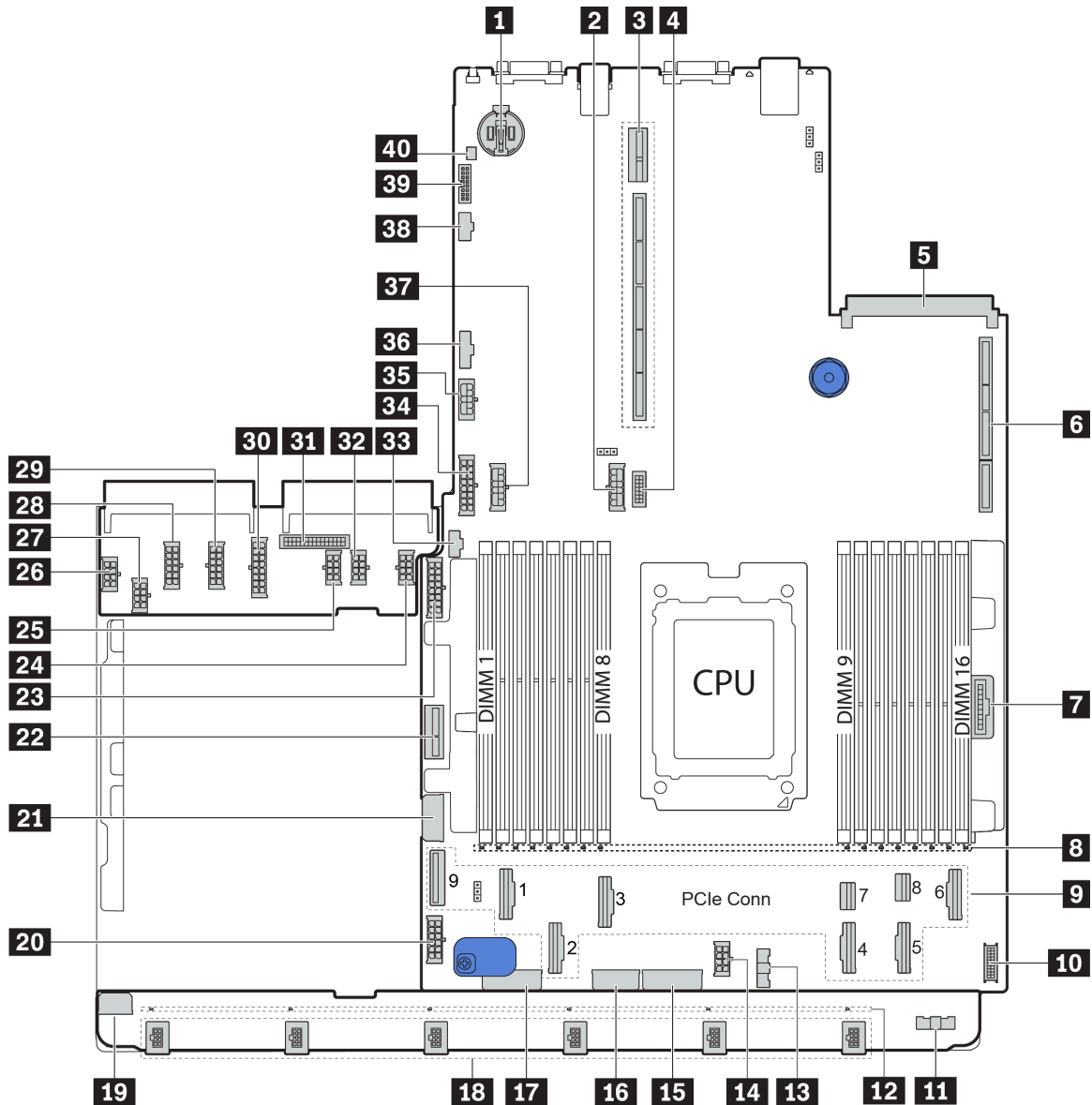
圖例 19. 主機板元件
