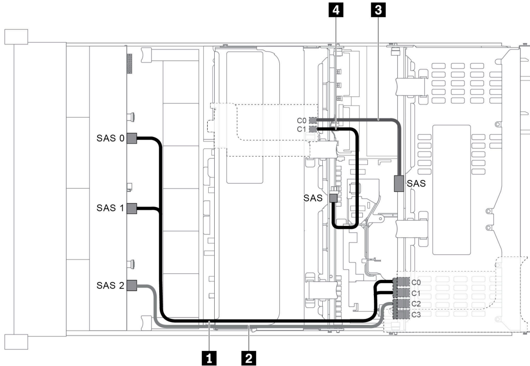
圖例 50. 配置為一個 12 x 3.5 吋 SAS/SATA 前方背板、一個背面框架、一個中間框架和兩張 RAID/HBA 配接卡 (8i+16i) 的纜線佈線
