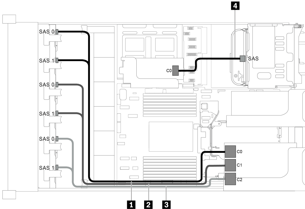
圖例 83. 配置為三個 8 x 2.5 吋 SAS/SATA 前方背板、一個後方框架和兩張 RAID/HBA 配接卡 (8i+32i) 的纜線佈線
