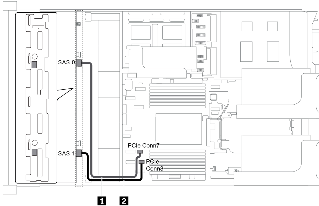
圖例 42. 配置為一個 8 x 3.5 吋 SAS/SATA 前方背板的纜線佈線
