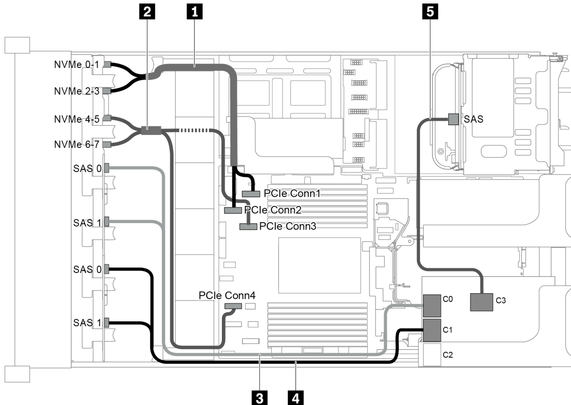
圖例 94. 配置為三個前方背板 (8 NVMe + 2 x 8 SAS/SATA)、一個後方框架和一張 32i RAID 配接卡的纜線佈線
