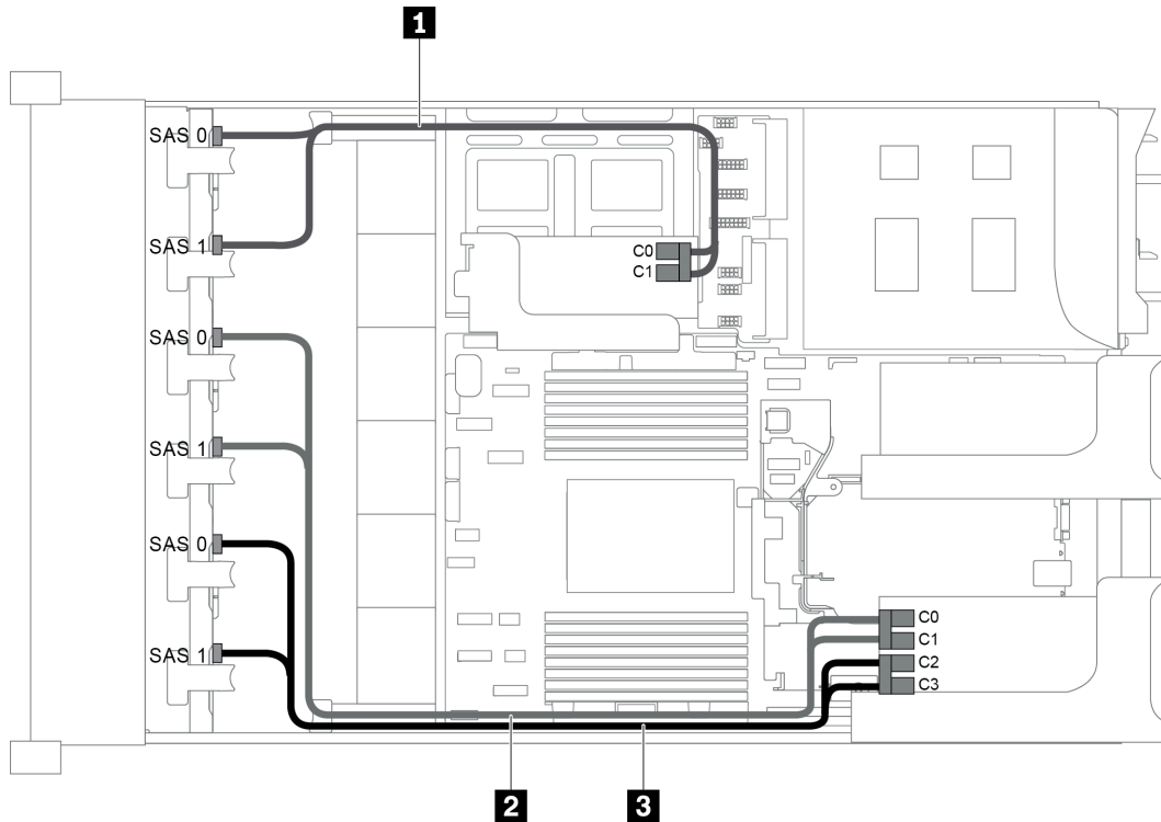
圖例 76. 配置為三個 8 x 2.5 吋 SAS/SATA 前方背板和兩張 RAID/HBA 配接卡 (8i+16i) 的纜線佈線
