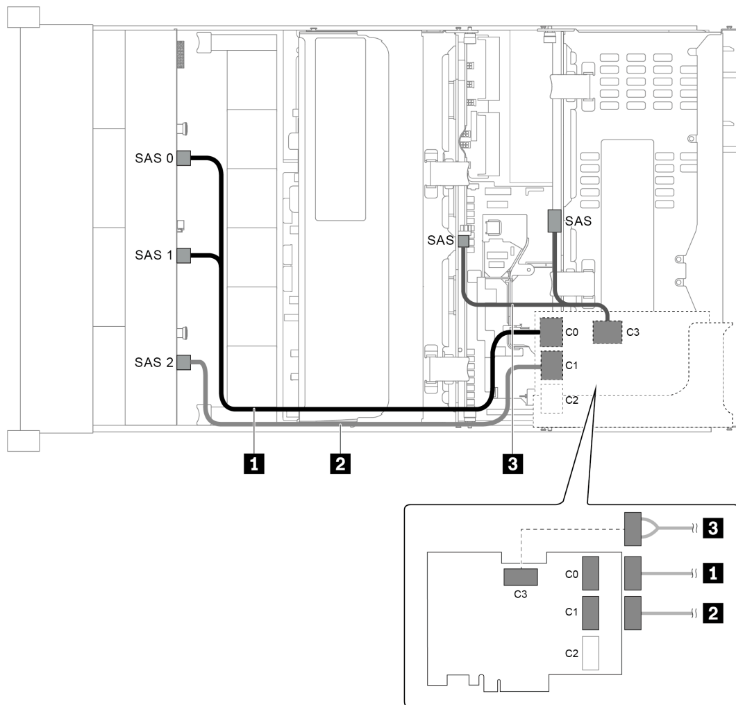
圖例 51. 配置為一個 12 x 3.5 吋 SAS/SATA 前方背板、一個後方框架、一個中間框架和一張 32i RAID 配接卡的纜線佈線
