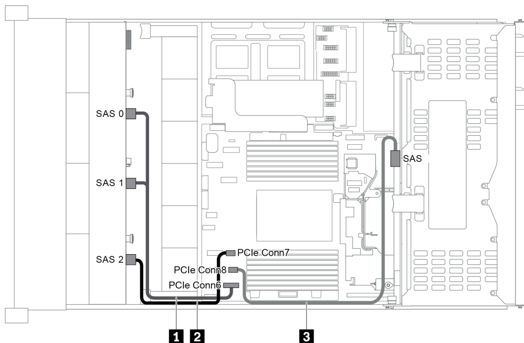
圖例 46. 配置為一個 12 x 3.5 吋 SAS/SATA 前方背板和一個背面框架 (SAS/SATA) 的纜線佈線
