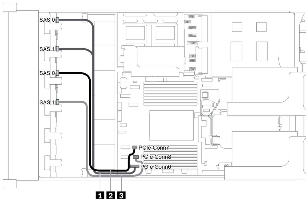
圖例 61. 配置為兩個 8 x 2.5 吋 SAS/SATA 前方背板的纜線佈線
