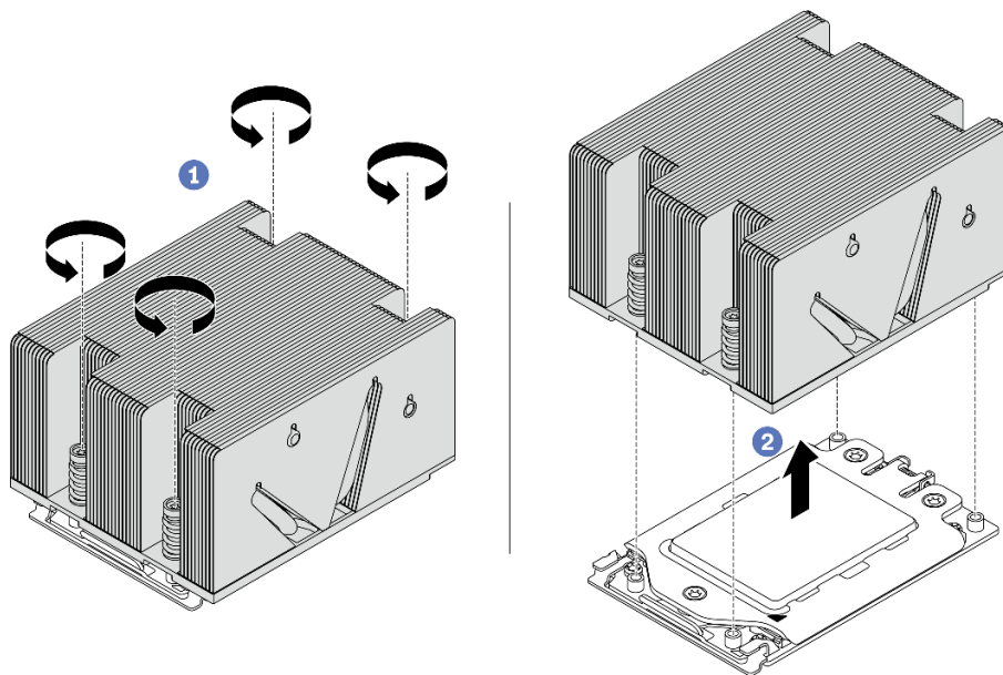
圖例 114. 卸下散熱槽
