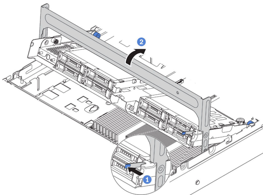
圖例 136. 關上框架把手
