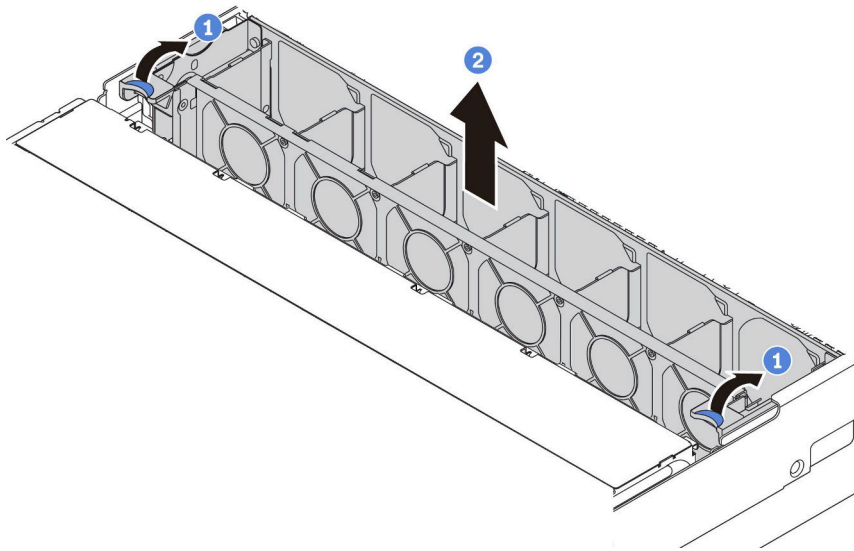
圖例 113. 卸下系統風扇機盒
