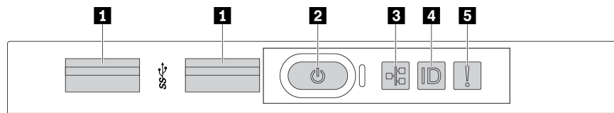
圖例 11. 配備八個 3.5 吋機槽之伺服器型號的正面 I/O 組件
