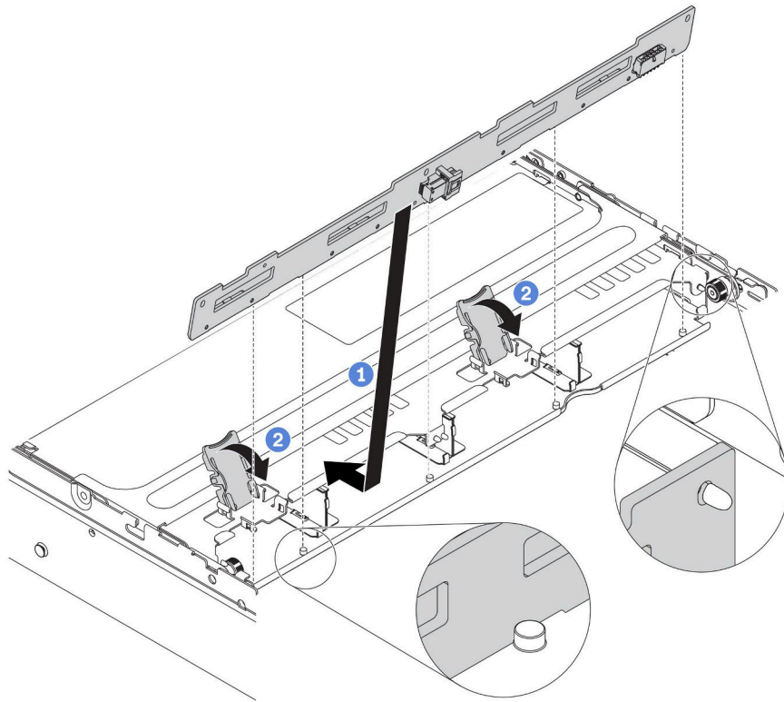
圖例 137. 安裝中間 3.5 吋硬碟背板
