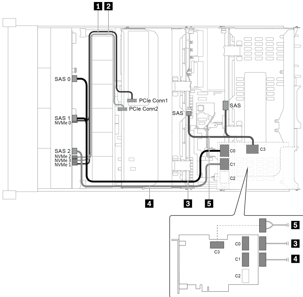
圖例 58. 配置為一個 12 x 3.5 吋 AnyBay 前方背板、一個後方框架、一個中間框架和一張 32i RAID 配接卡的纜線佈線
