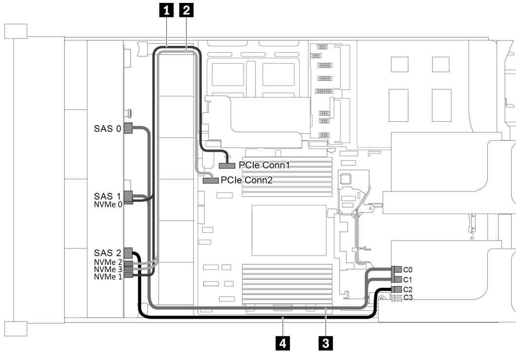
圖例 53. 配置為一個 12 x 3.5 吋 AnyBay 前方背板和一張 16i RAID/HBA 配接卡的纜線佈線
