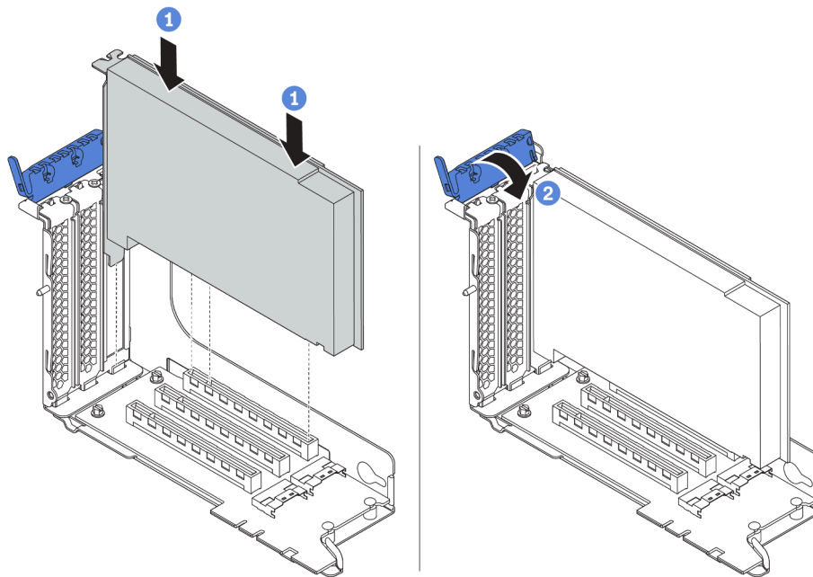
圖例 141. PCIe 配接卡安裝
