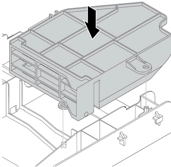
圖例 143. 安裝單倍寬 GPU 配接卡適用的 GPU 空氣擋板附加元件
