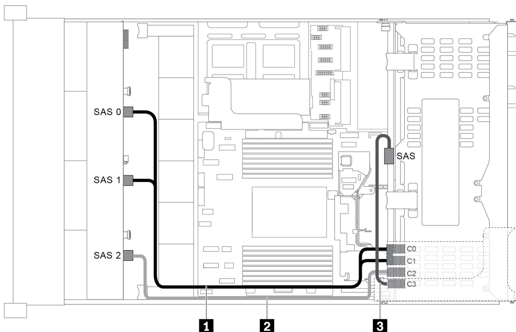
圖例 47. 配置為一個 12 x 3.5 吋 SAS/SATA 前方背板、一個背面框架和一張 16i RAID/HBA 配接卡的纜線佈線
