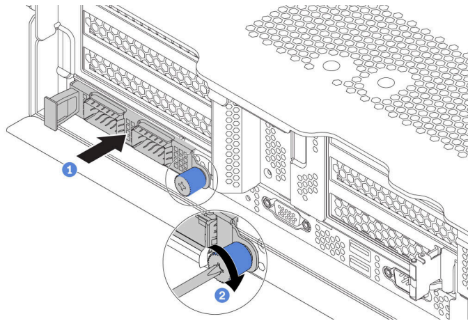
圖例 150. OCP 3.0 乙太網路配接卡安裝
