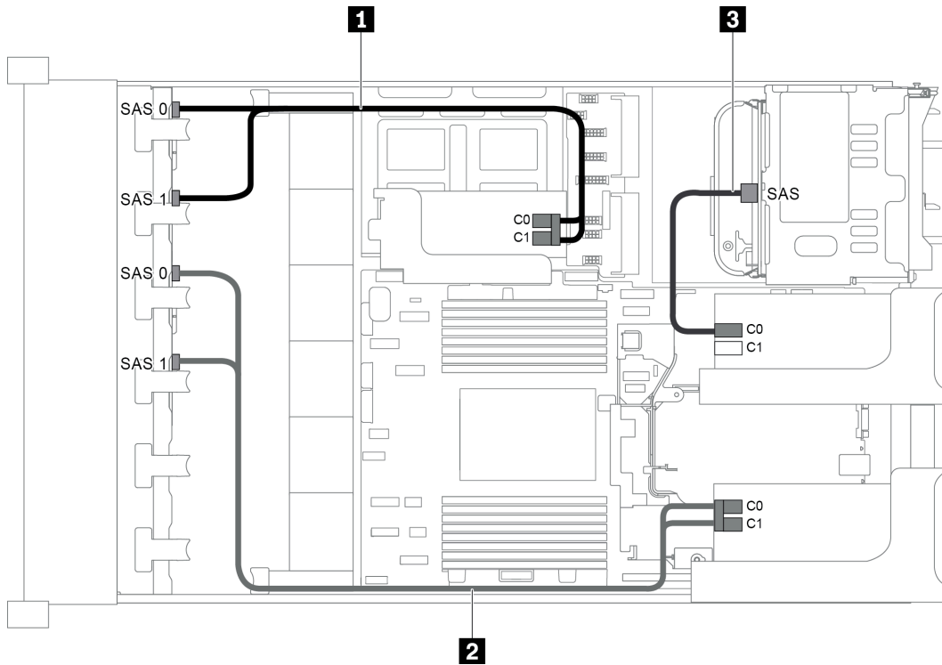
圖例 66. 配置為兩個 8 x 2.5 吋 SAS/SATA 前方背板、一個後方框架和三張 8i RAID/HBA 配接卡的纜線佈線
