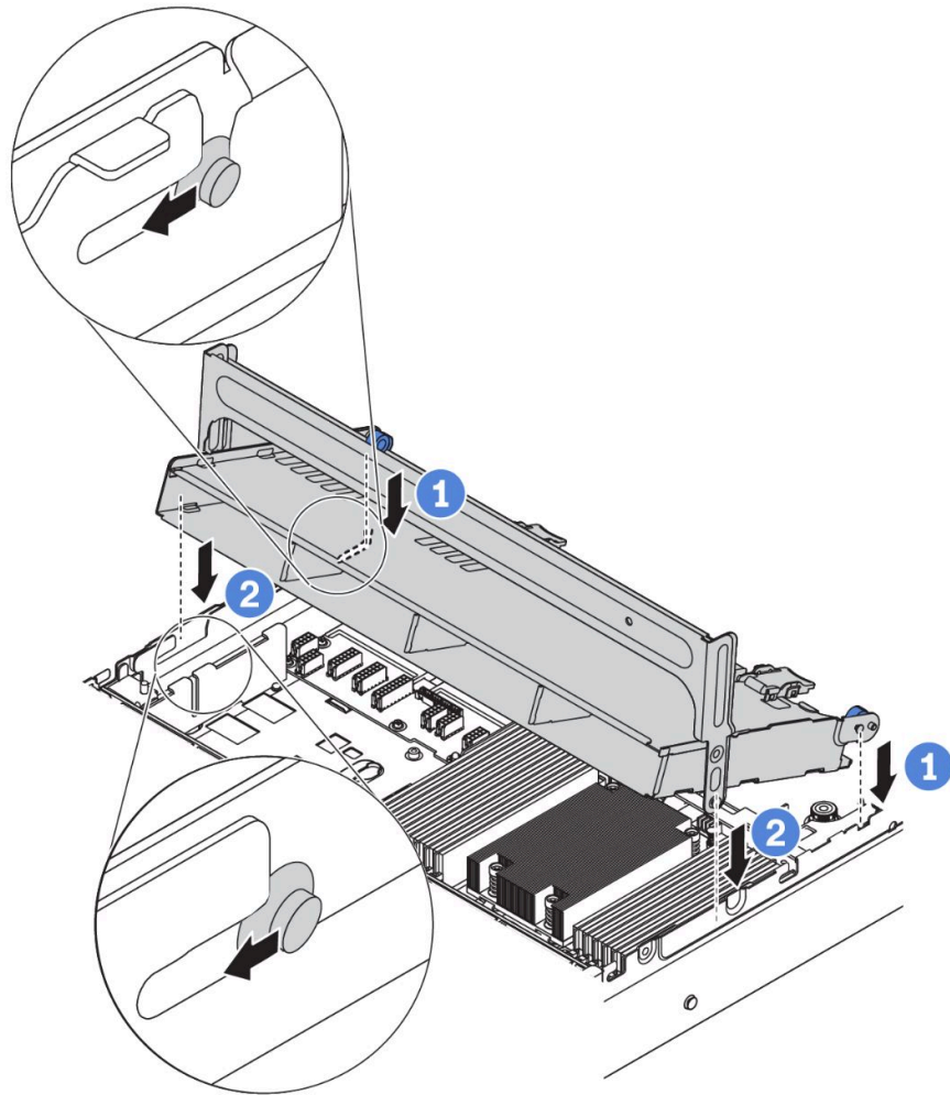
圖例 138. 安裝中間 3.5 吋框架
