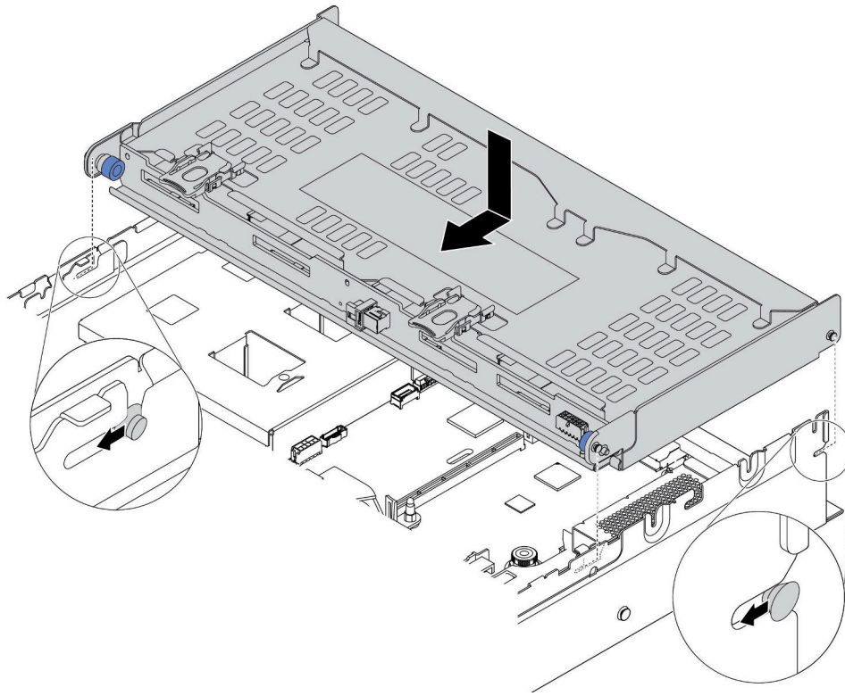
圖例 149. 安裝背面 3.5 吋框架
