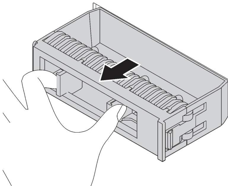
圖例 159. 卸下 3.5 吋硬碟填充板
