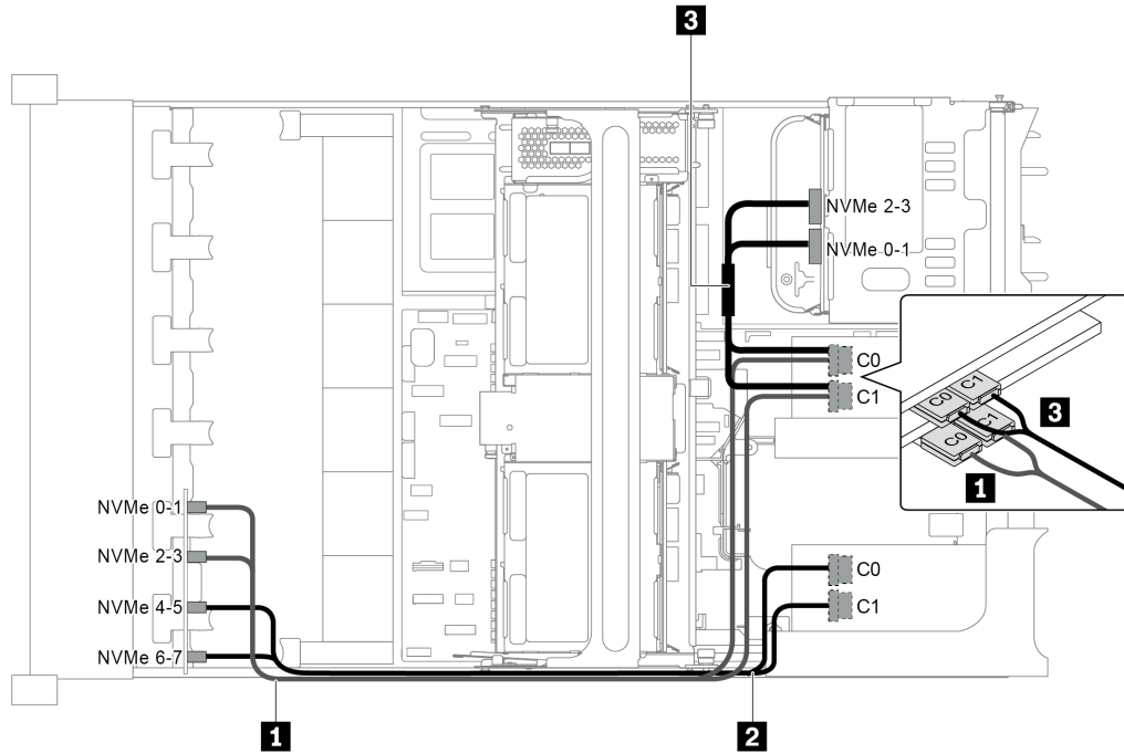
圖例 105. 配置為三個 NVMe 重定時器配接卡 (一個在後方背板上，兩個在前方背板上) 的纜線佈線
