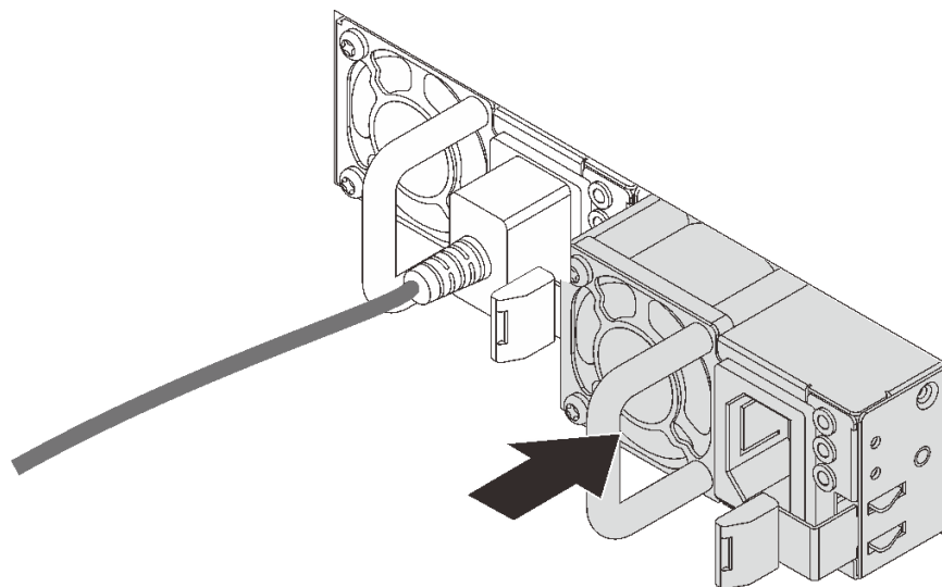
圖例 157. 安裝熱抽換電源供應器
