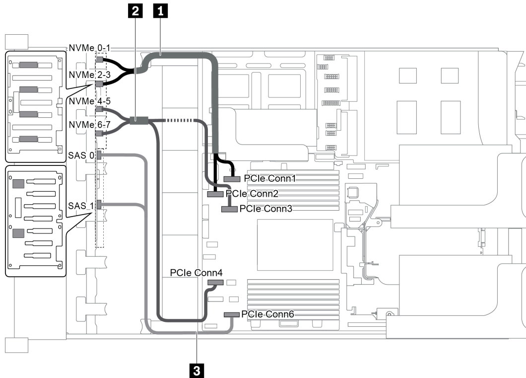
圖例 68. 配置為兩個前方背板 (8 NVMe + 8 SAS/SATA) 的纜線佈線
