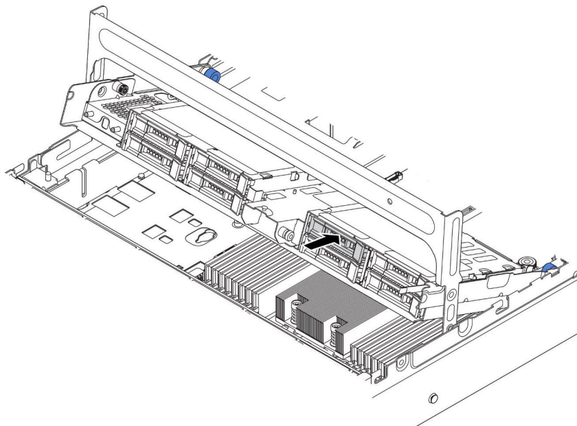
圖例 135. 將硬碟裝入框架
