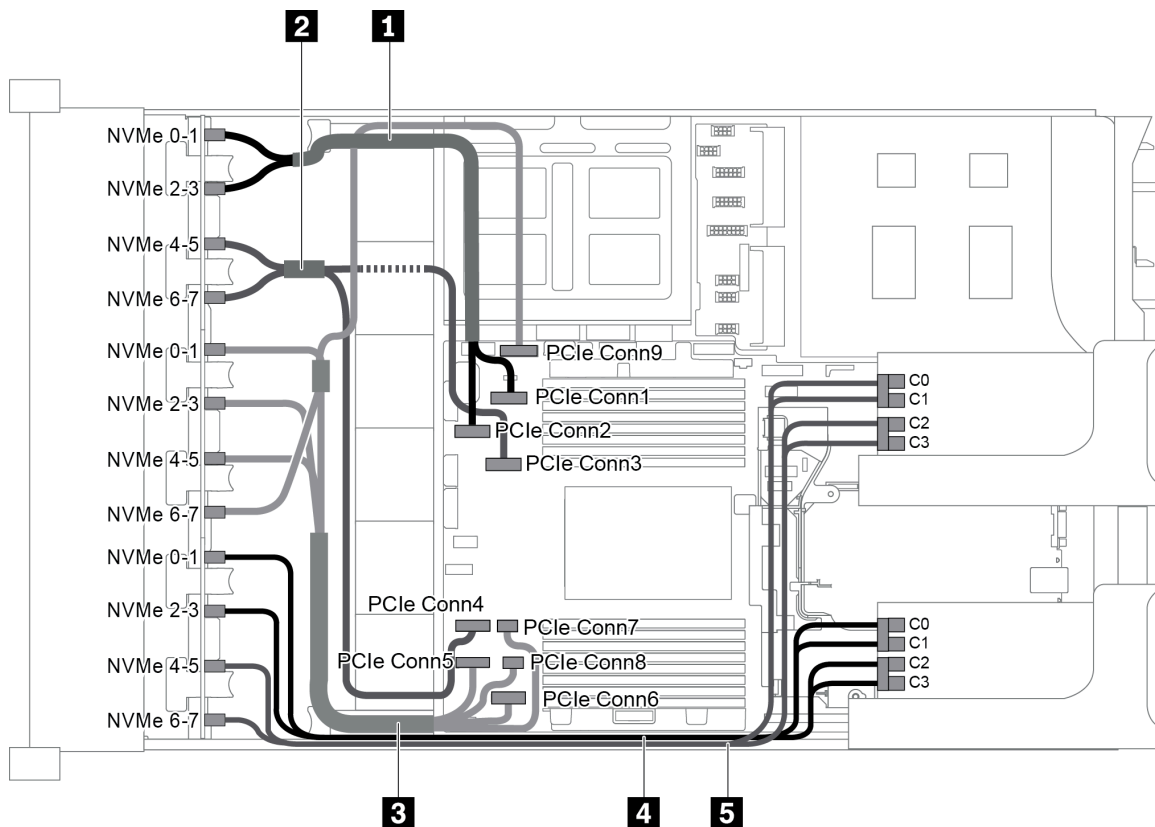
圖例 96. 配置為三個 8 x 2.5 吋 NVMe 前方背板和兩張 810-4P 或 1610-4P NVMe 交換器卡的纜線佈線
