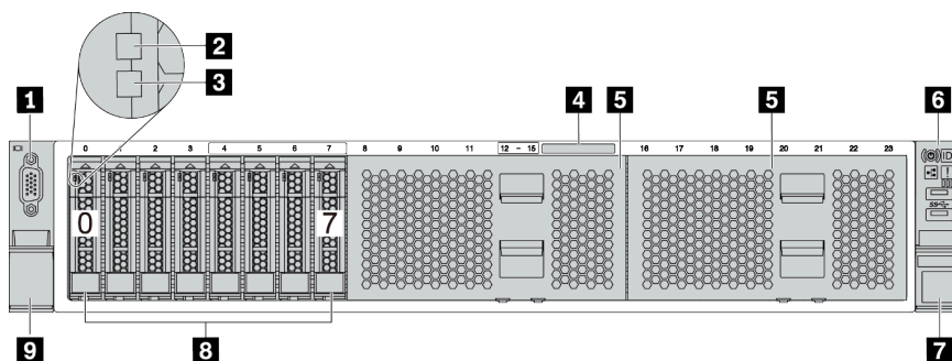
圖例 5. 配備八個 2.5 吋機槽的伺服器型號
