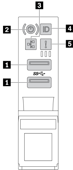
圖例 12. 配備 2.5 吋機槽或十二個 3.5 吋機槽之伺服器型號的正面 I/O 組件
