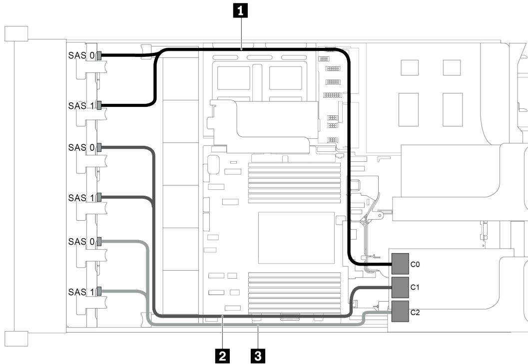
圖例 82. 配置為三個 8 x 2.5 吋 SAS/SATA 前方背板和一張 32i RAID 配接卡的纜線佈線
