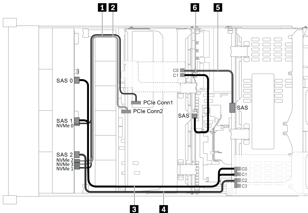
圖例 57. 配置為一個 12 x 3.5 吋 AnyBay 前方背板、一個後方框架、一個中間框架和兩張 RAID/HBA 配接卡 (8i+16i) 的纜線佈線
