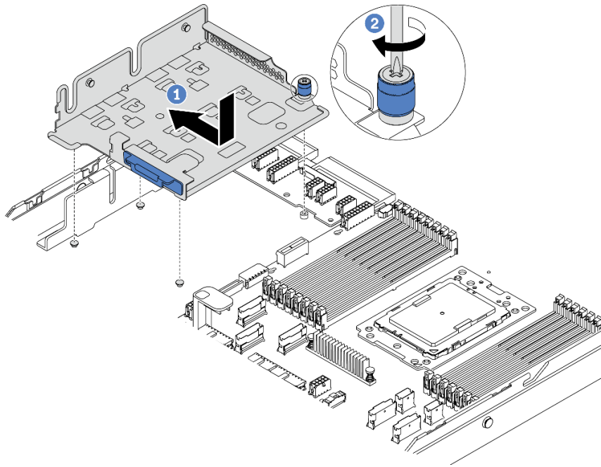
圖例 117. 支撐托架安裝
