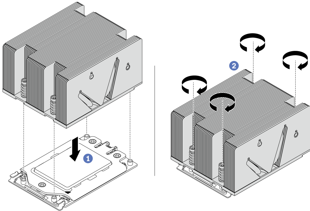
圖例 115. 安裝散熱槽
