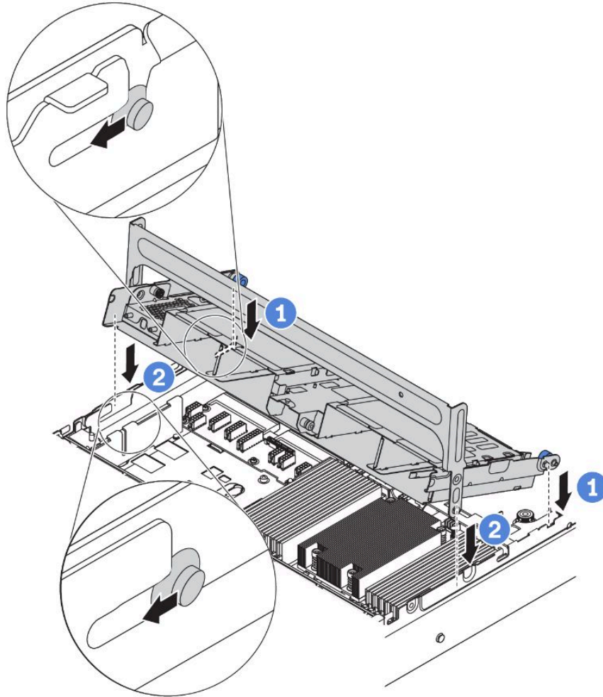
圖例 134. 安裝中間 2.5 吋框架
