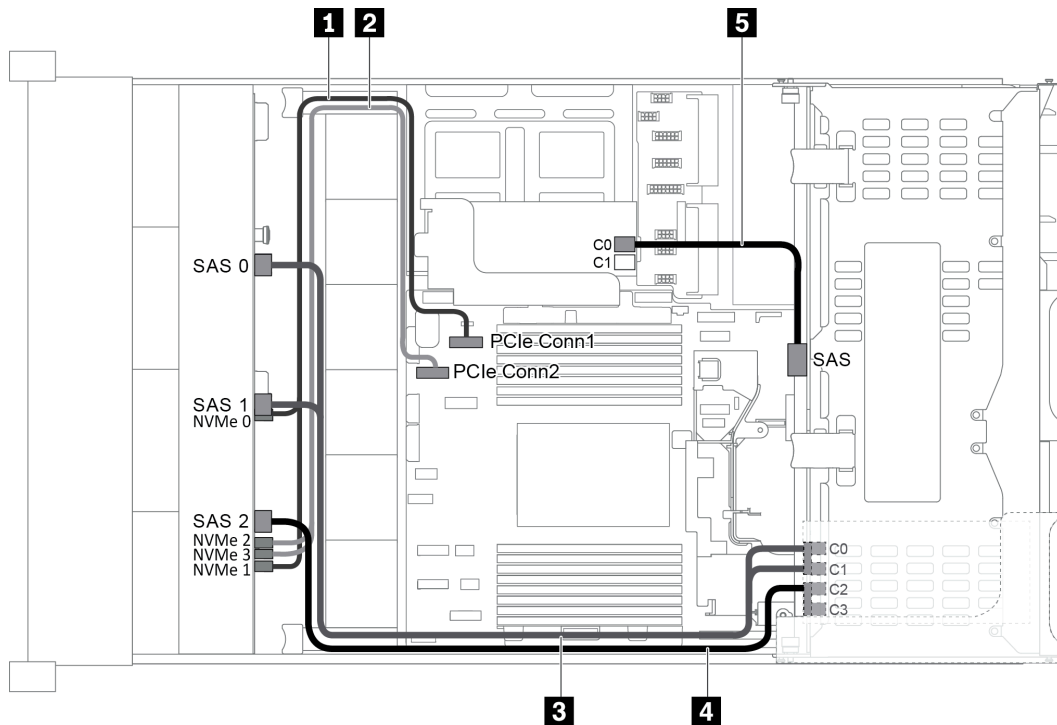
圖例 55. 配置為一個 12 x 3.5 吋 AnyBay 前方背板、一個後方框架和兩張 RAID/HBA 配接卡的纜線佈線 (8i+16i)
