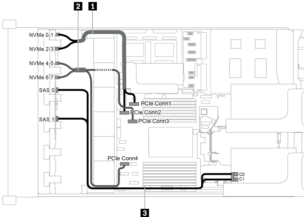
圖例 69. 配置為兩個前方背板 (8 NVMe + 8 SAS/SATA) 和一張 8i RAID/HBA 配接卡的纜線佈線
