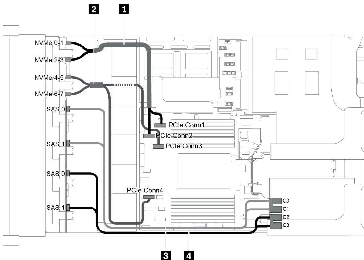
圖例 86. 配置為三個前方背板 (8 NVMe + 2 x 8 SAS/SATA) 和一張 16i RAID/HBA 配接卡的纜線佈線
