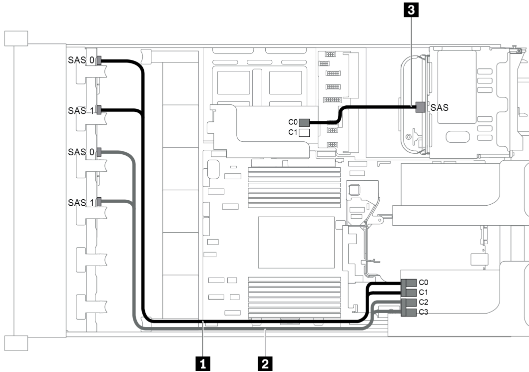
圖例 65. 配置為兩個 8 x 2.5 吋 SAS/SATA 前方背板、一個背面框架和兩張 RAID/HBA 配接卡 (8i+16i) 的纜線佈線
