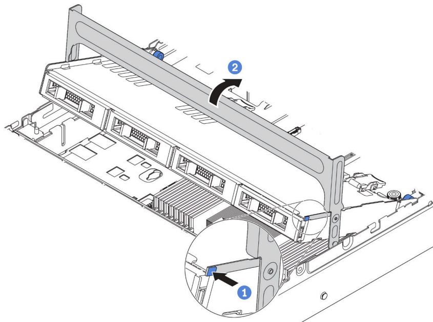
圖例 140. 關上框架把手
