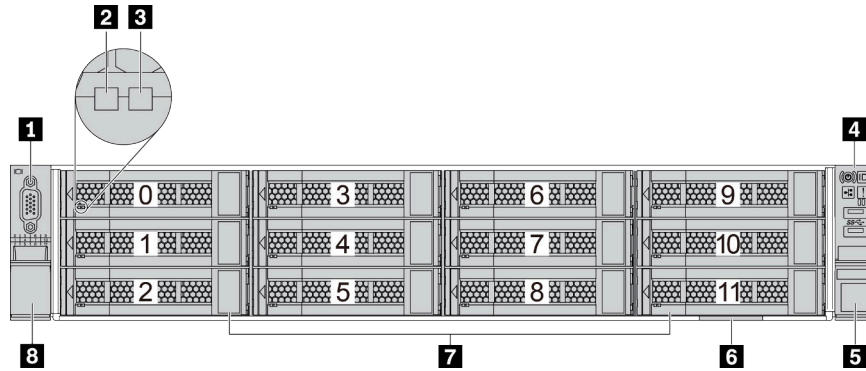
圖例 9. 配備十二個 3.5 吋機槽的伺服器型號
