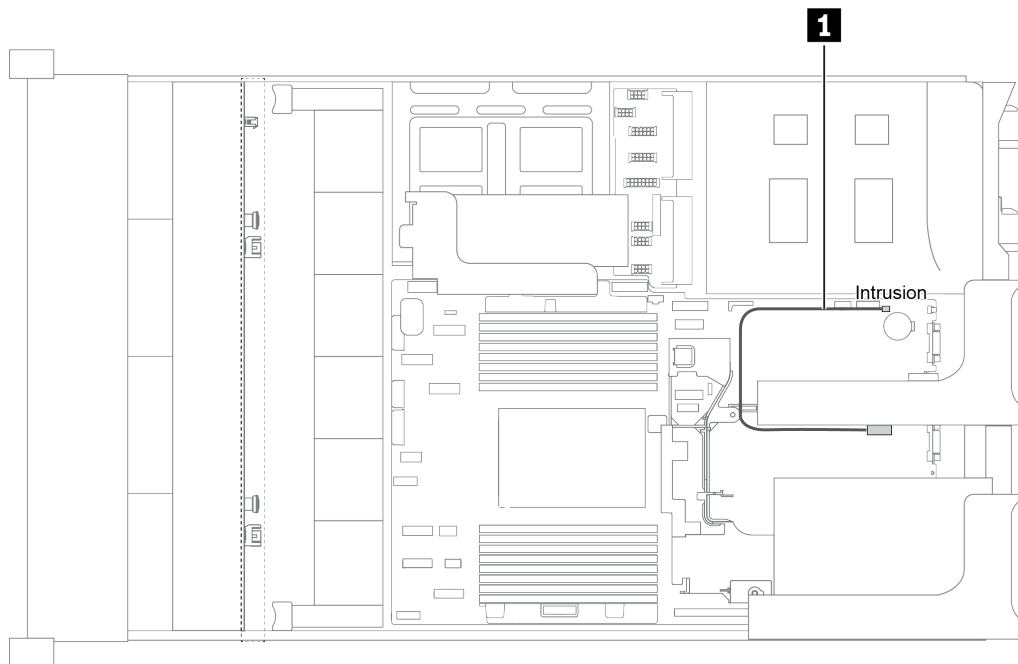
圖例 31. 入侵開關纜線佈線
