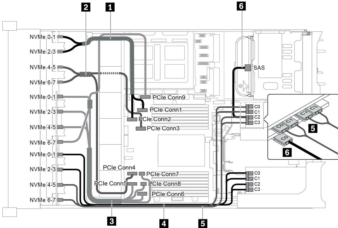
圖例 98. 配置為三個 8 x 2.5 吋 NVMe 前方背板、一個背面框架 (SAS/SATA)、兩張 810-4P 或 1610-4P NVMe 交換器卡和一張 8i RAID/HBA 配接卡的纜線佈線
