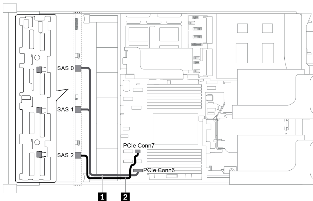
圖例 44. 配置為一個 12 x 3.5 吋 SAS/SATA 前方背板的纜線佈線
