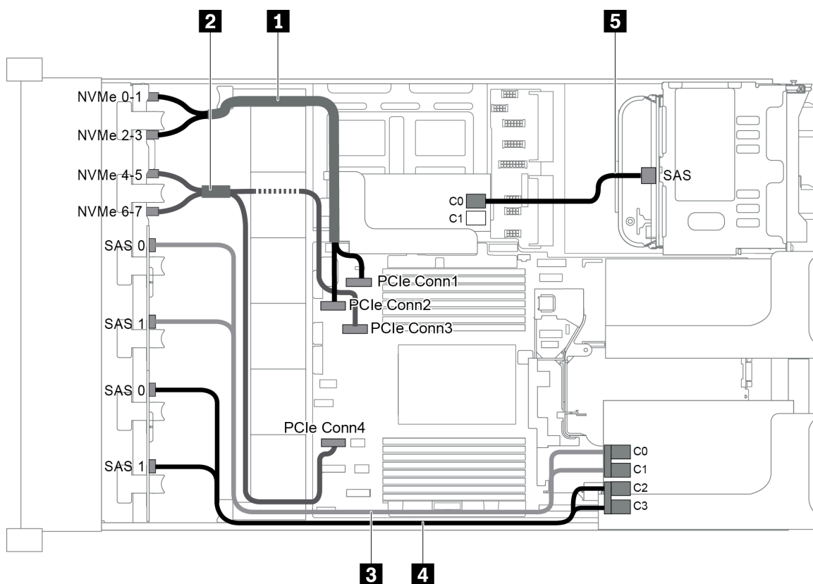
圖例 89. 配置為三個前方背板 (8 NVMe + 2 x 8 SAS/SATA)、一個背面框架和兩張 RAID/HBA 配接卡 (8i+16i) 的纜線佈線
