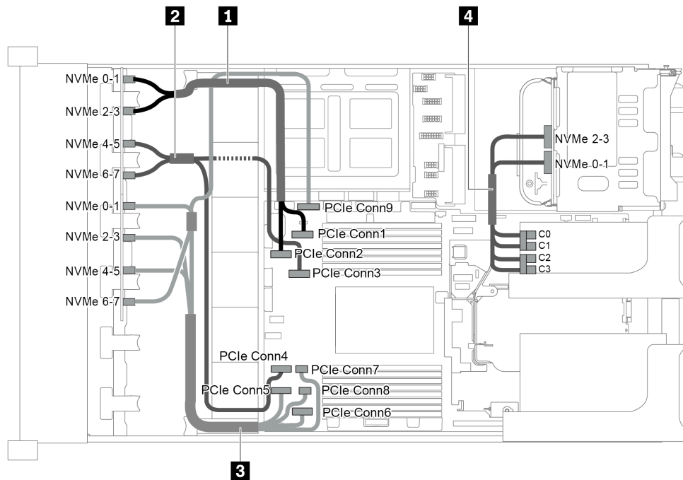
圖例 74. 配置為兩個 8 x 2.5 吋 NVMe 前方背板、一個背面框架 (NVMe) 和一張 810-4P 或 1610-4P NVMe 交換器卡的纜線佈線
