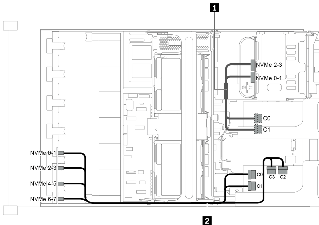
圖例 106. 配置為後方背板上的一個 NVMe 重定時器配接卡和一個 1611-8P NVMe 交換器卡的纜線佈線
