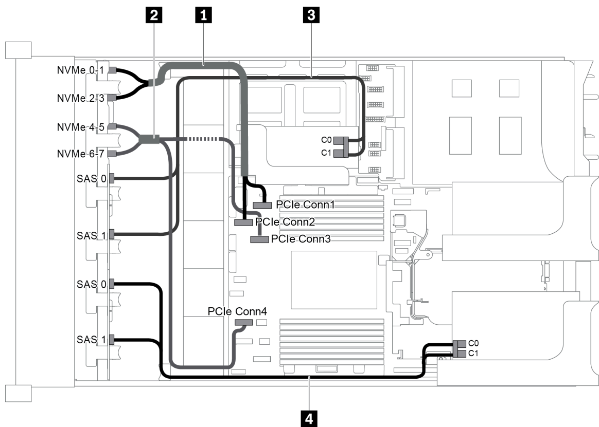
圖例 87. 配置為三個前方背板 (8 NVMe + 2 x 8 SAS/SATA) 和兩張 8i RAID/HBA 配接卡的纜線佈線
