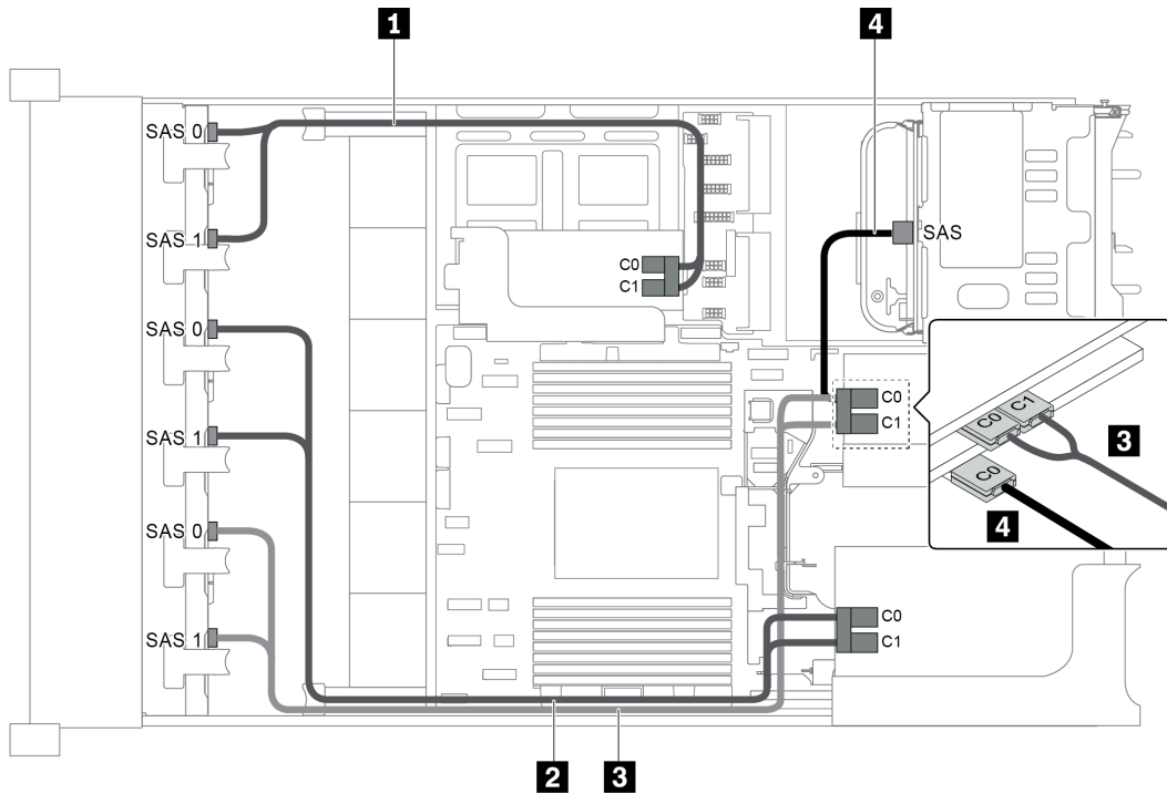
圖例 79. 配置為三個 8 x 2.5 吋 SAS/SATA 前方背板、一個後方框架和四張 8i RAID/HBA 配接卡的纜線佈線
