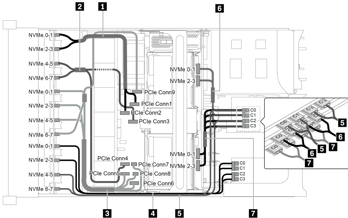
圖例 101. 配置為三個 8 x 2.5 吋 NVMe 前方背板、一個中間框架 (NVMe) 和四張 810-4P 或 1610-4P NVMe 交換器卡的纜線佈線
