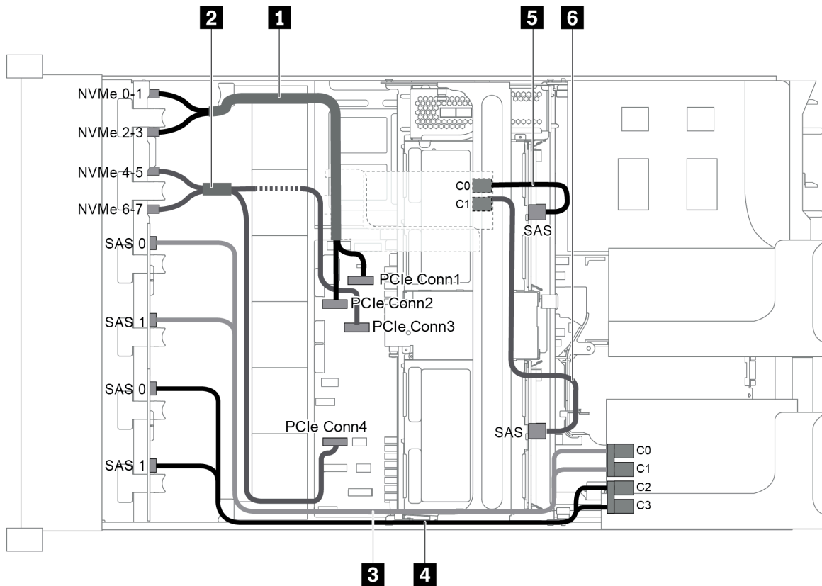
圖例 92. 配置為三個前方背板 (8 NVMe + 2 x 8 SAS/SATA)、一個中間框架和兩張 RAID/HBA 配接卡 (8i+16i) 的纜線佈線
