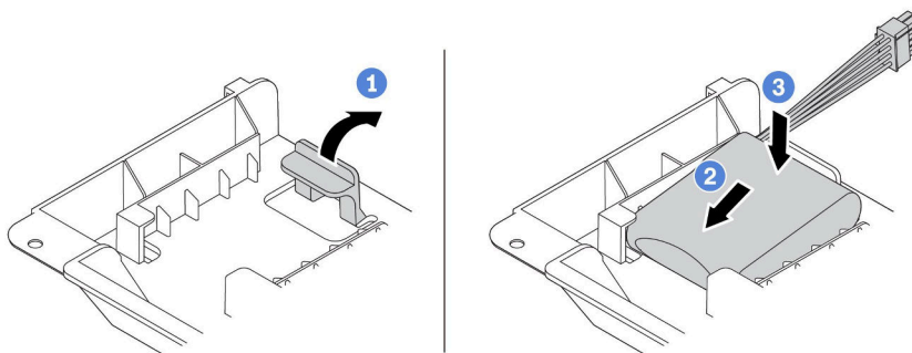
圖例 120. 空氣擋板上的超級電容器安裝
