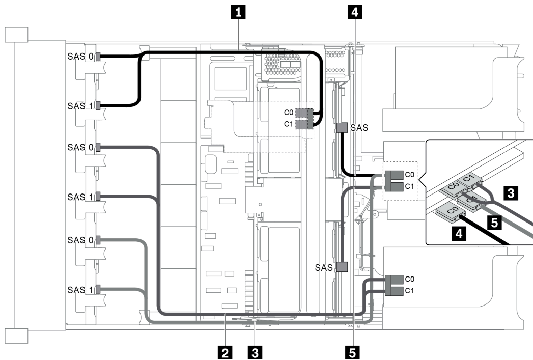
圖例 81. 配置為三個 8 x 2.5 吋 SAS/SATA 前方背板、一個中間框架和四張 8i RAID/HBA 配接卡的纜線佈線
