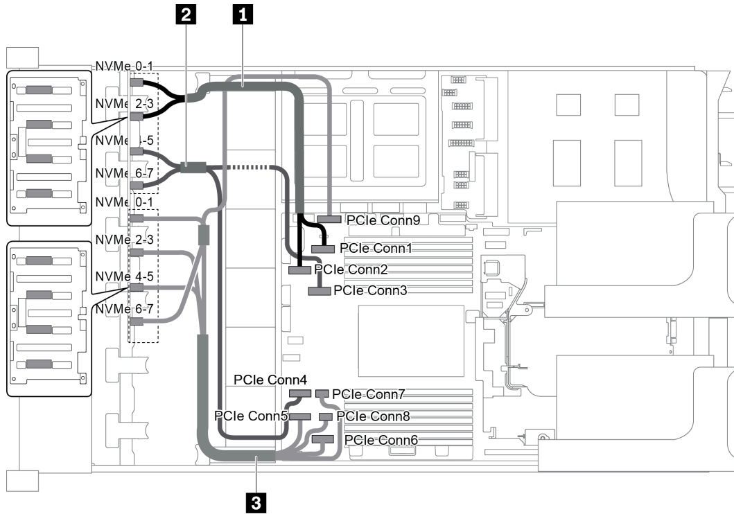
圖例 72. 配置為兩個 8 x 2.5 吋 NVMe 前方背板的纜線佈線
