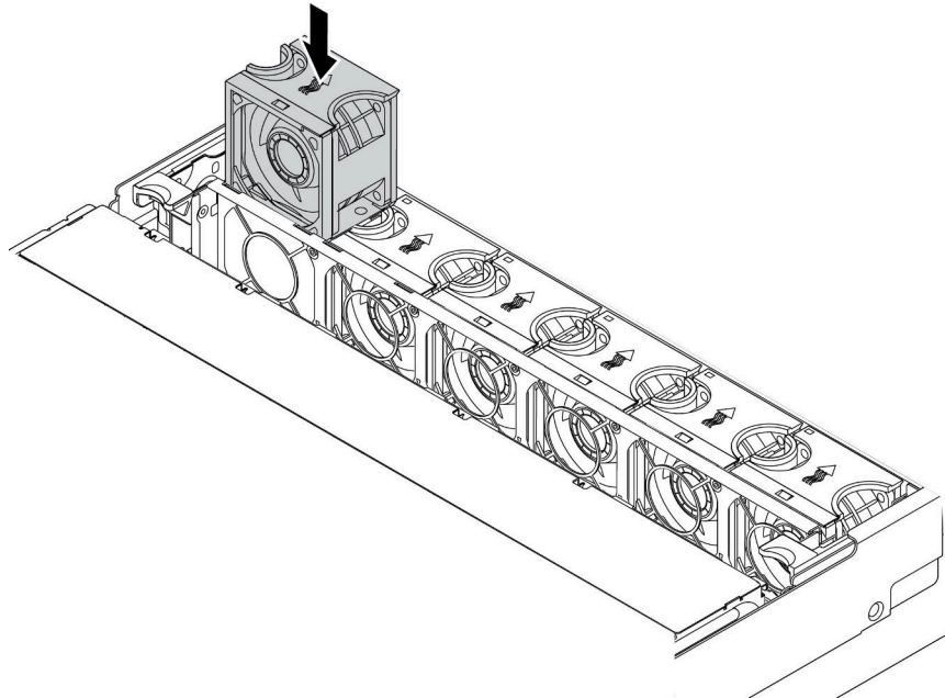
圖例 132. 安裝系統風扇
