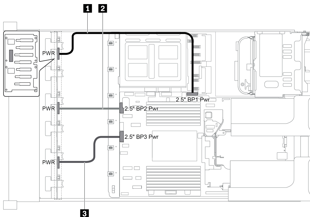
圖例 36. 前方 2.5 吋硬碟背板的電源佈線
