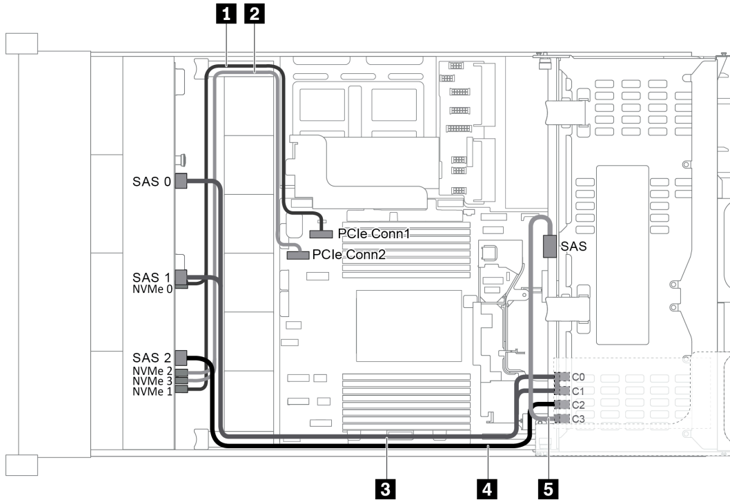
圖例 54. 配置為一個 12 x 3.5 吋 AnyBay 前方背板、一個後方框架和一張 16i RAID/HBA 配接卡的纜線佈線
