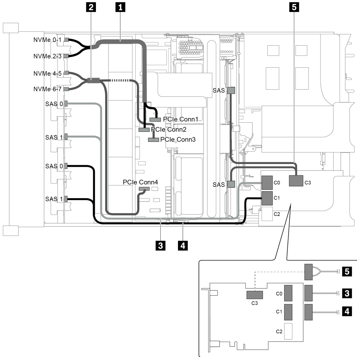
圖例 95. 配置為三個前方背板 (8 NVMe + 2 x 8 SAS/SATA)、一個中間框架和一張 32i RAID 配接卡的纜線佈線
