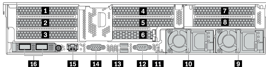
圖例 13. 具有八個 PCIe 插槽之伺服器型號的背面圖
