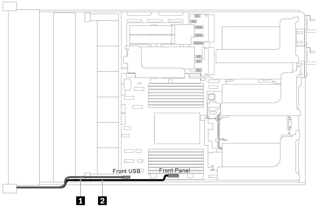
圖例 24. 右機架門鎖上正面 I/O 組件的纜線佈線
