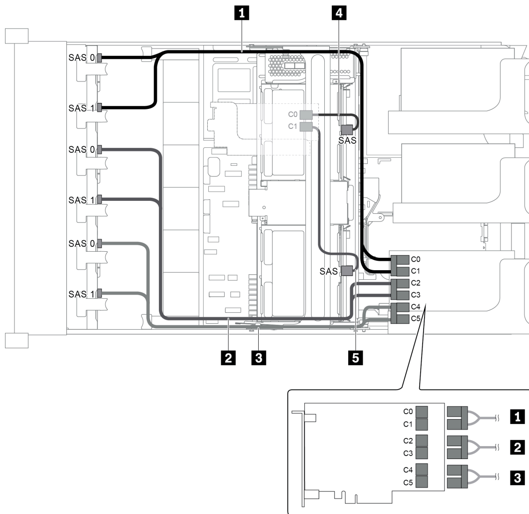
圖例 80. 配置為三個 8 x 2.5 吋 SAS/SATA 前方背板、一個中間框架和兩張 RAID/HBA 配接卡 (8i+24i) 的纜線佈線
