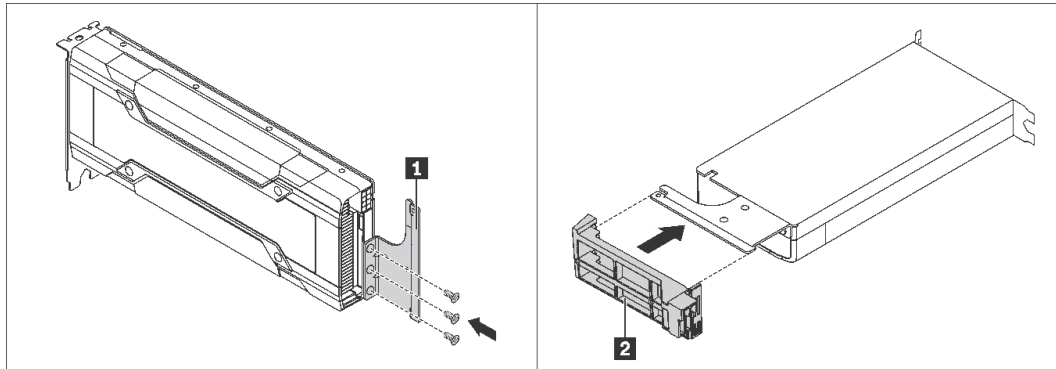
圖例 142. 安裝雙寬 GPU 配接卡適用的 GPU 空氣擋板附加元件
