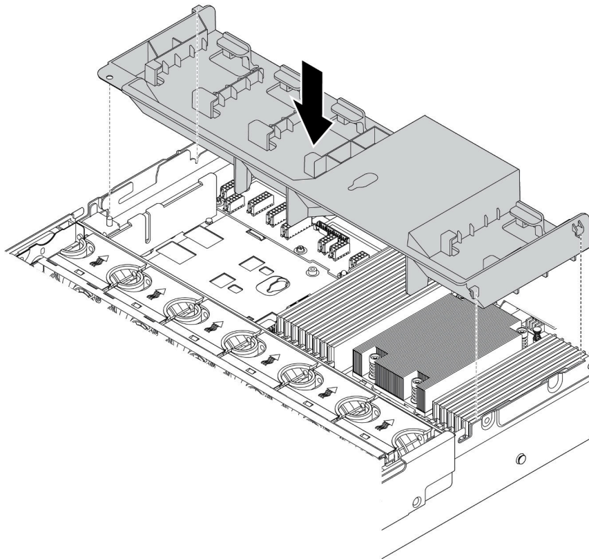
圖例 153. 安裝標準空氣擋板
