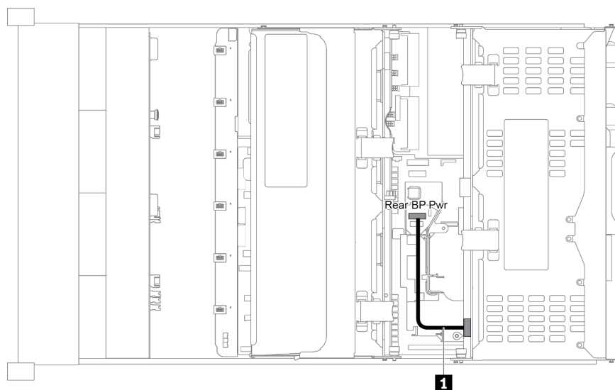
圖例 41. 後方 3.5 吋硬碟背板的電源佈線
