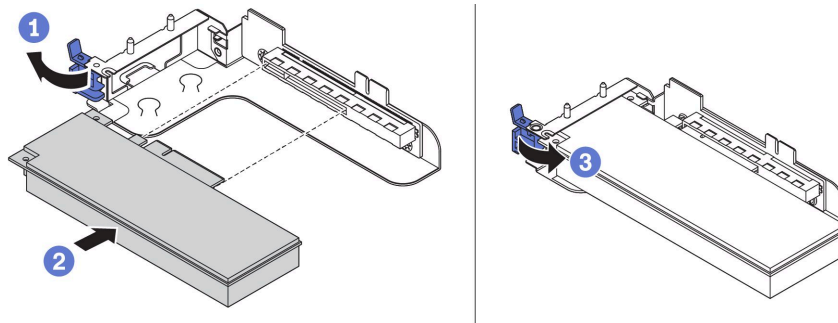
圖例 122. PCIe 配接卡安裝
