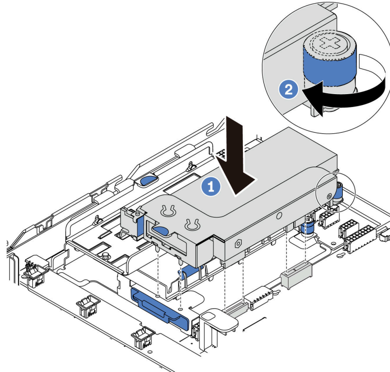
圖例 123. 內部擴充卡組件安裝
