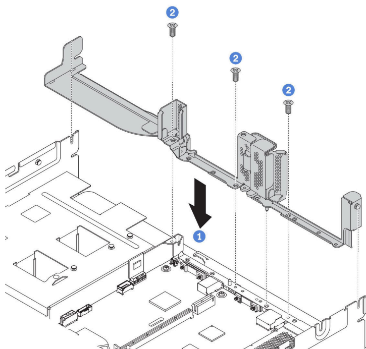
圖例 144. 安裝背面 2.5 吋框架的後壁托架
