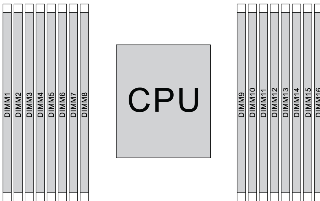
圖例 108. DIMM 位置
