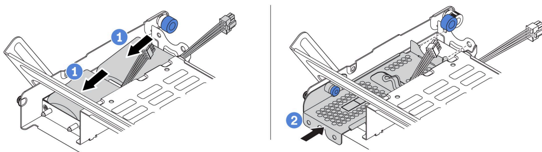
圖例 121. 中間 2.5 吋框架上的超級電容器安裝
