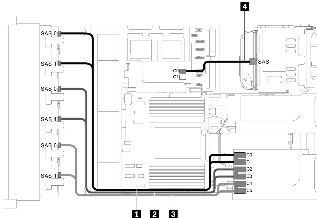
圖例 78. 配置為三個 8 x 2.5 吋 SAS/SATA 前方背板、一個背面框架和兩張 RAID/HBA 配接卡 (8i+24i) 的纜線佈線
