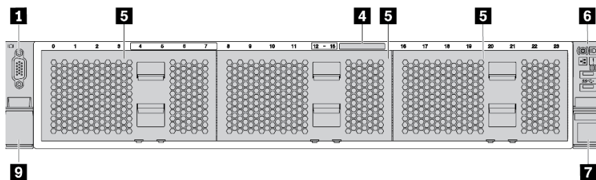
圖例 4. 未配備背板之伺服器型號
