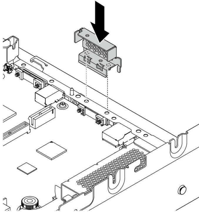
圖例 147. 安裝背面 3.5 吋框架的後壁托架
