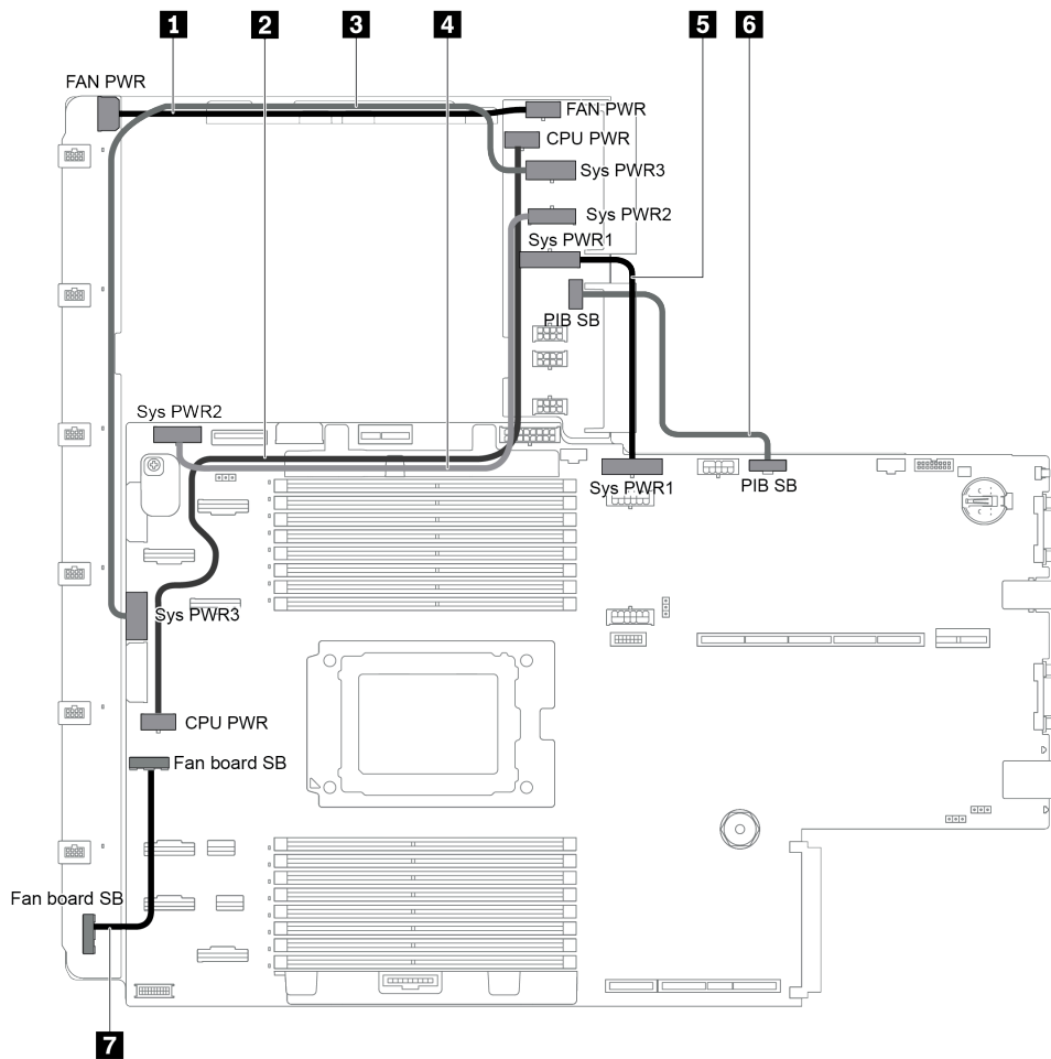
圖例 107. 主機板、PIB 板和風扇板之間的連線
