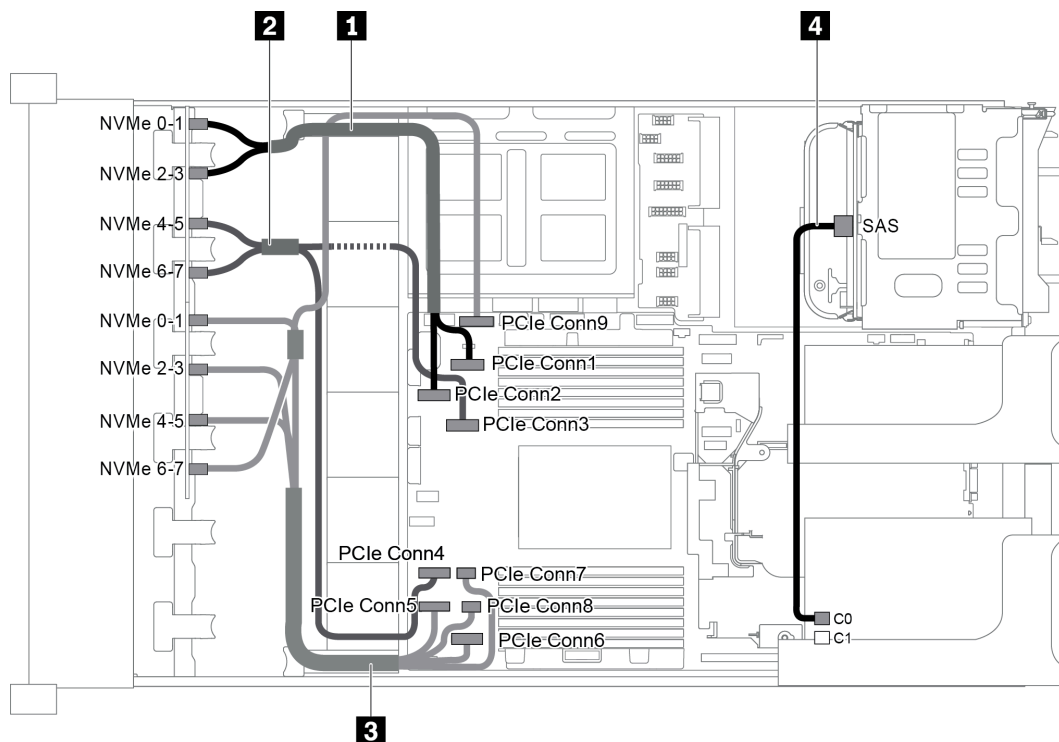
圖例 73. 配置為兩個 8 x 2.5 吋 NVMe 前方背板、一個背面框架 (SAS/SATA) 和一張 8i RAID/HBA 配接卡的纜線佈線
