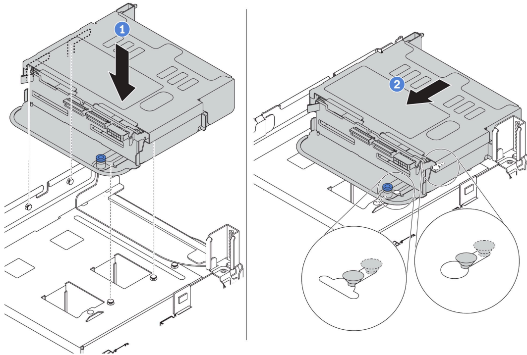
圖例 146. 安裝背面 2.5 吋框架
