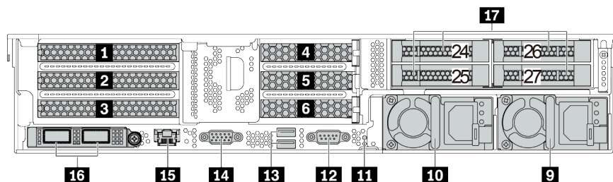
圖例 14. 配備 2.5 吋背面機槽和六個 PCIe 插槽之伺服器型號的背面圖
