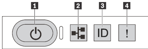
Abbildung 15. Anzeigen an der vorderen Bedienerkonsole
