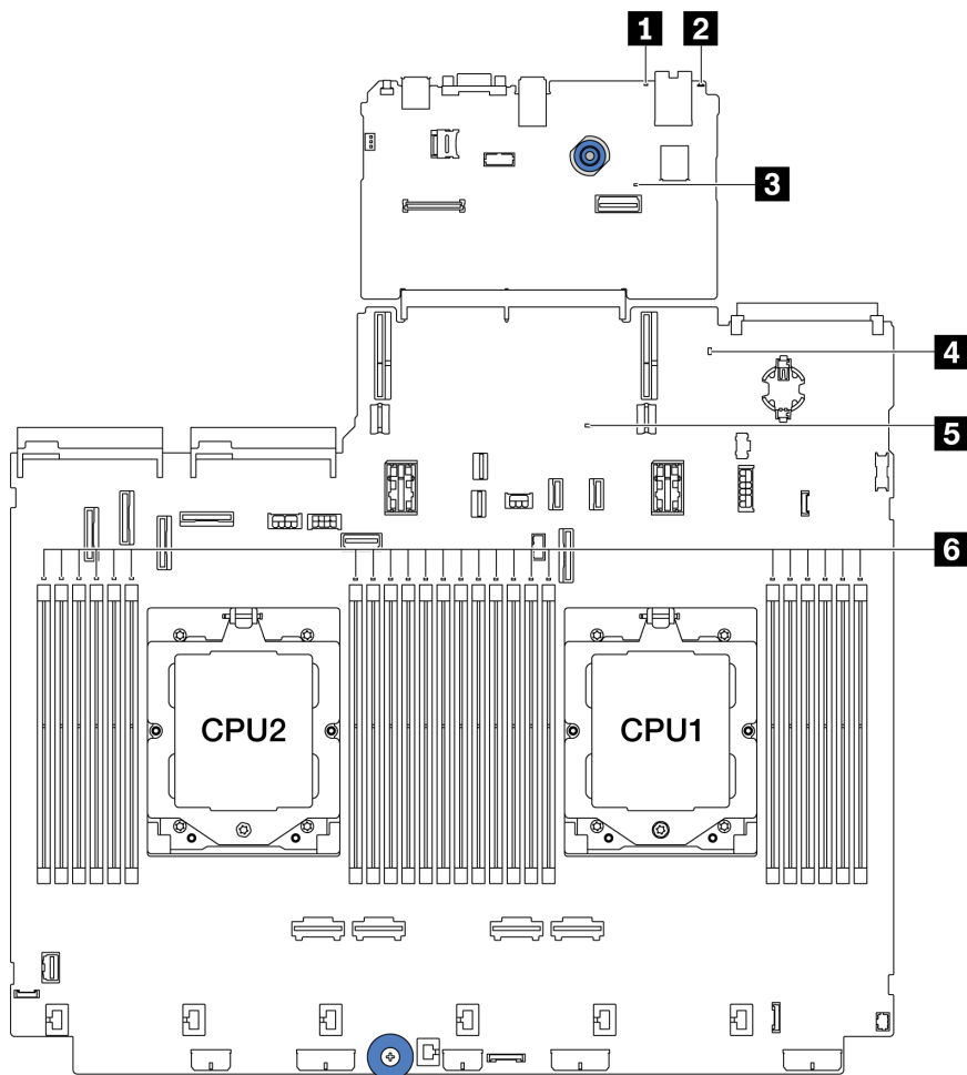
Abbildung 19. Anzeigen an der Systemplatinenbaugruppe
