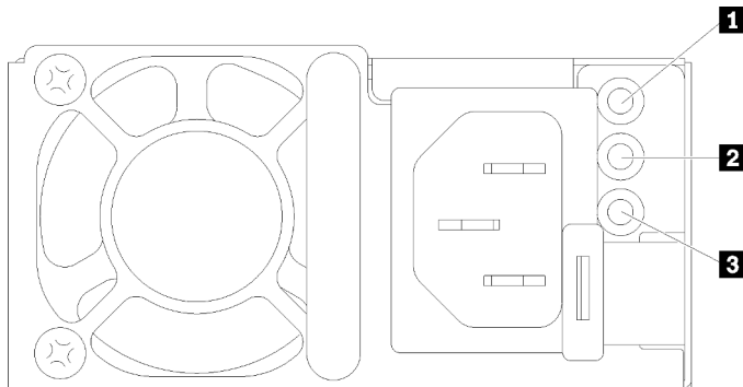
Abbildung 18. Netzteilanzeigen
