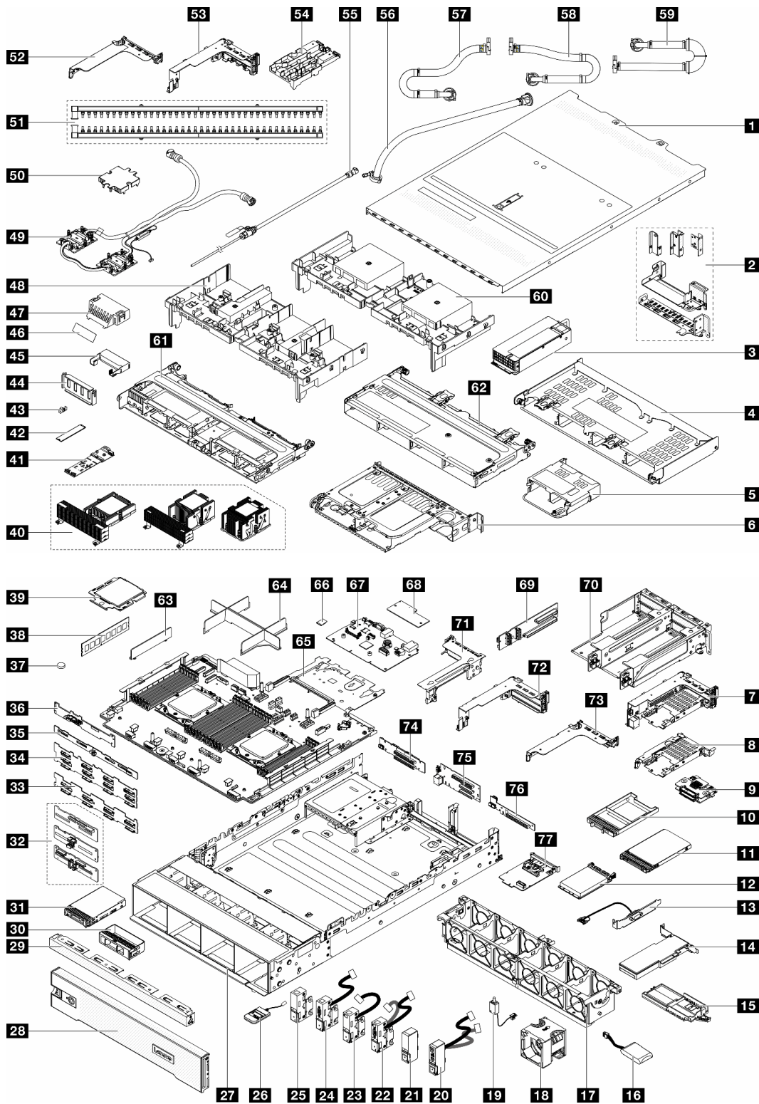
Abbildung 22. Serverkomponenten (Gehäuse mit 3,5-Zoll-Laufwerkpositionen)
