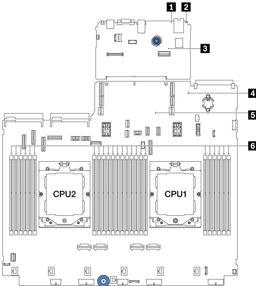
Figura 19. LED del conjunto de la placa del sistema
