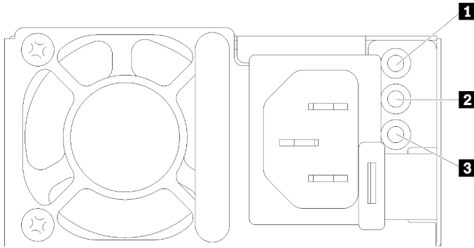
Figura 18. LED de la fuente de alimentación
