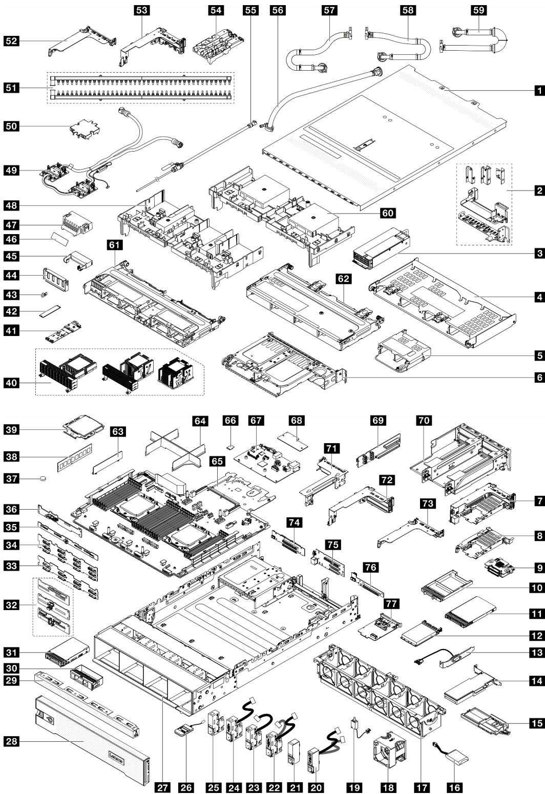
Figura 22. Componentes del servidor (chasis de bahía de unidad de 3,5")
